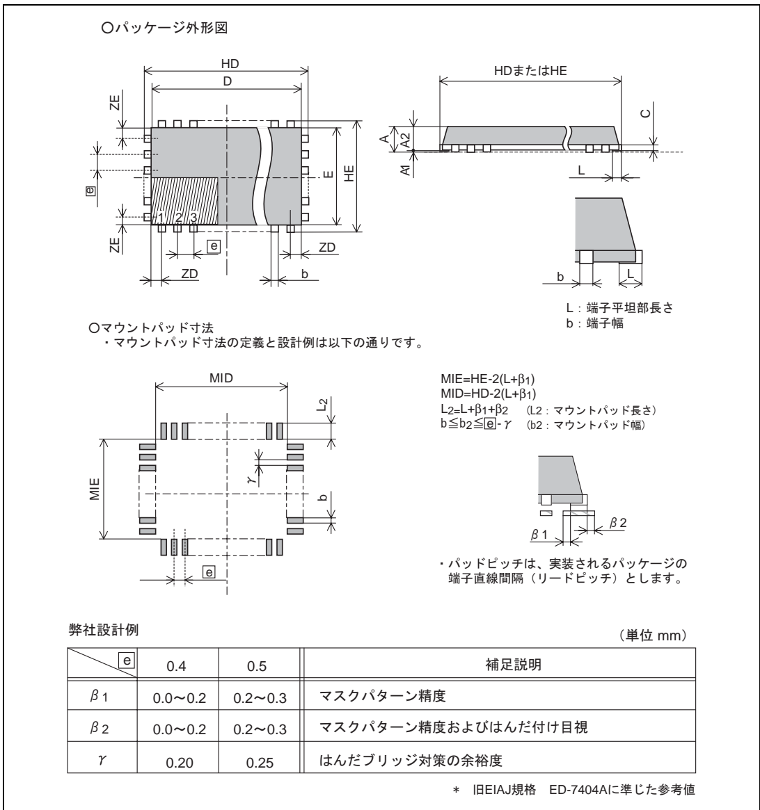
図 3.5 マウントパッド設計例
