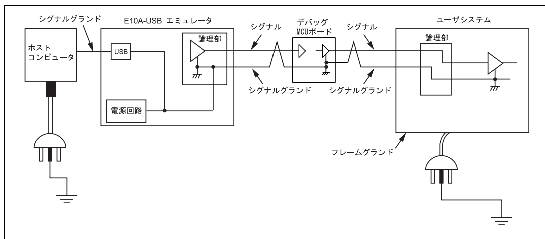
図 2.11 システムグランド系の接続
