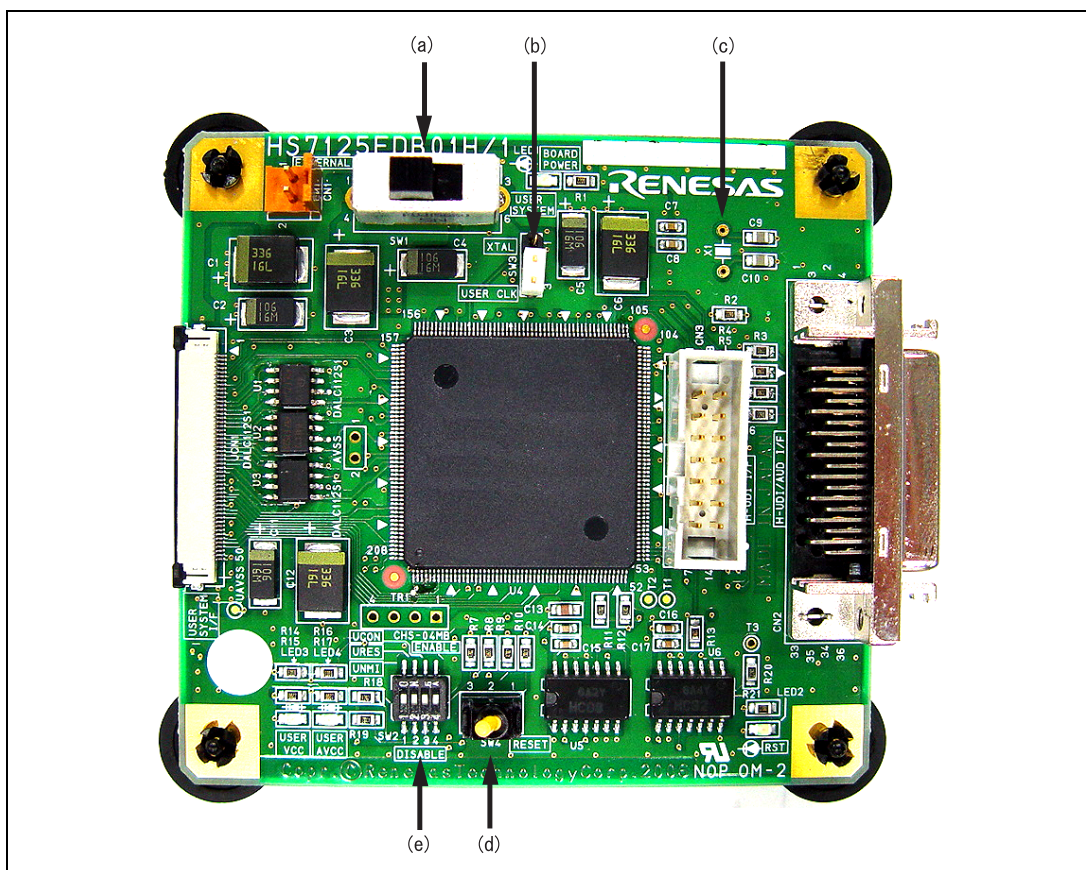
図 1.4 デバッグ MCU ボード本体の上面(2)
