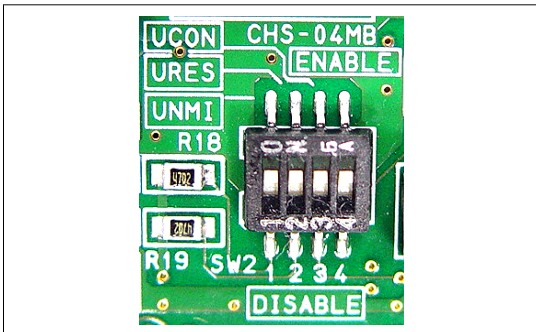
図 2.10 ユーザシステム入力信号有効/無効スイッチ
