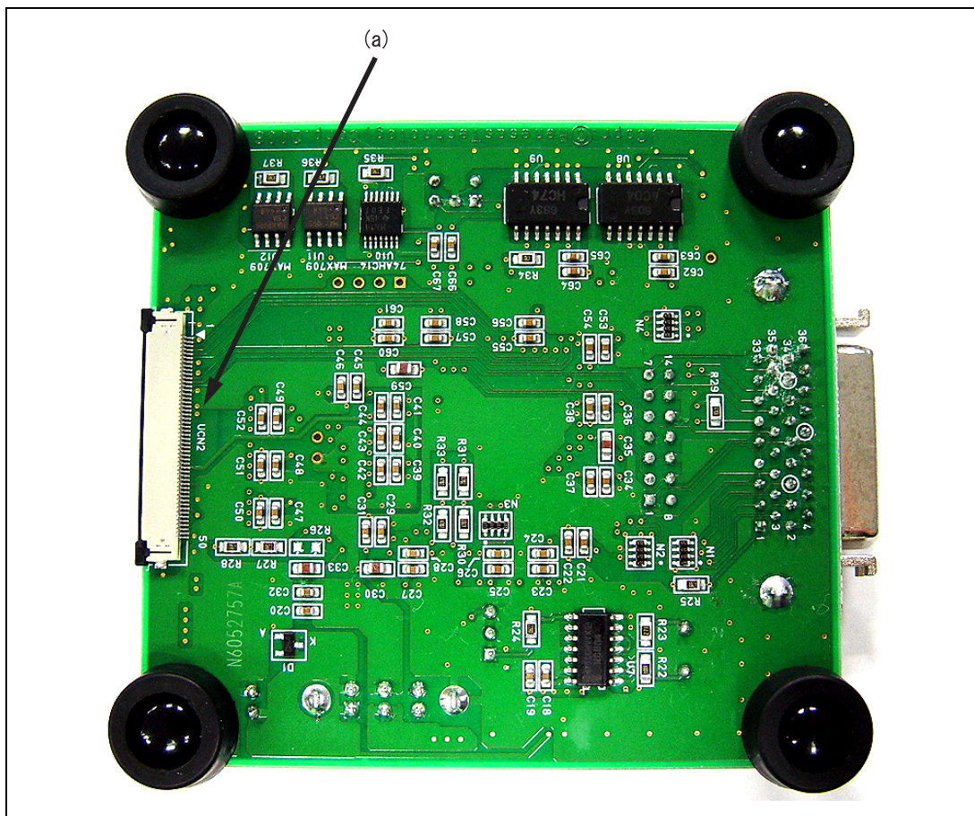
図 1.6 デバッグ MCU ボード本体の下面
