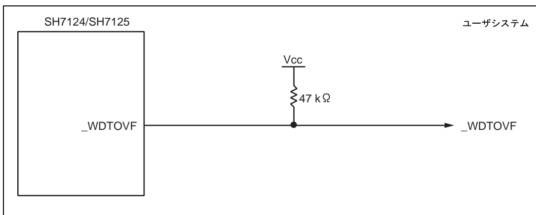
図 3.8 ユーザインタフェース回路(2)
