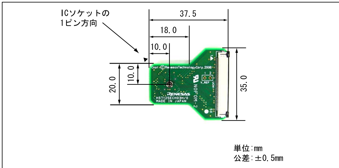
図 3.3 ユーザシステムインタフェースボードの外形寸法図
