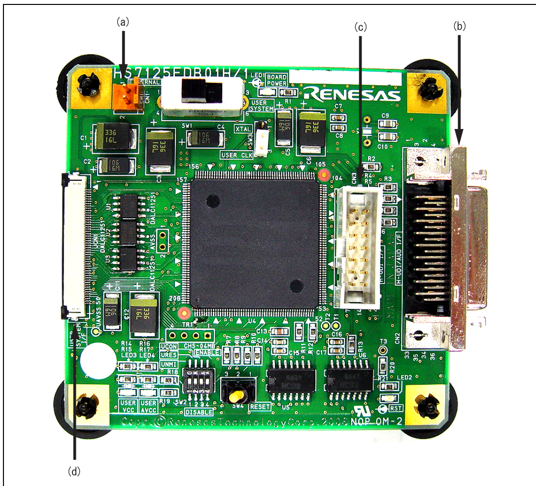
図 1.5 デバッグ MCU ボード本体の上面(3)
