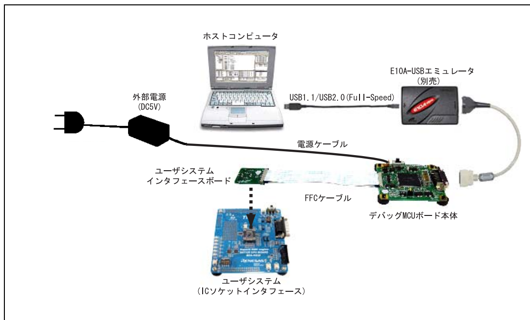
図 1.2 デバッグ MCU ボードのハードウェア構成
