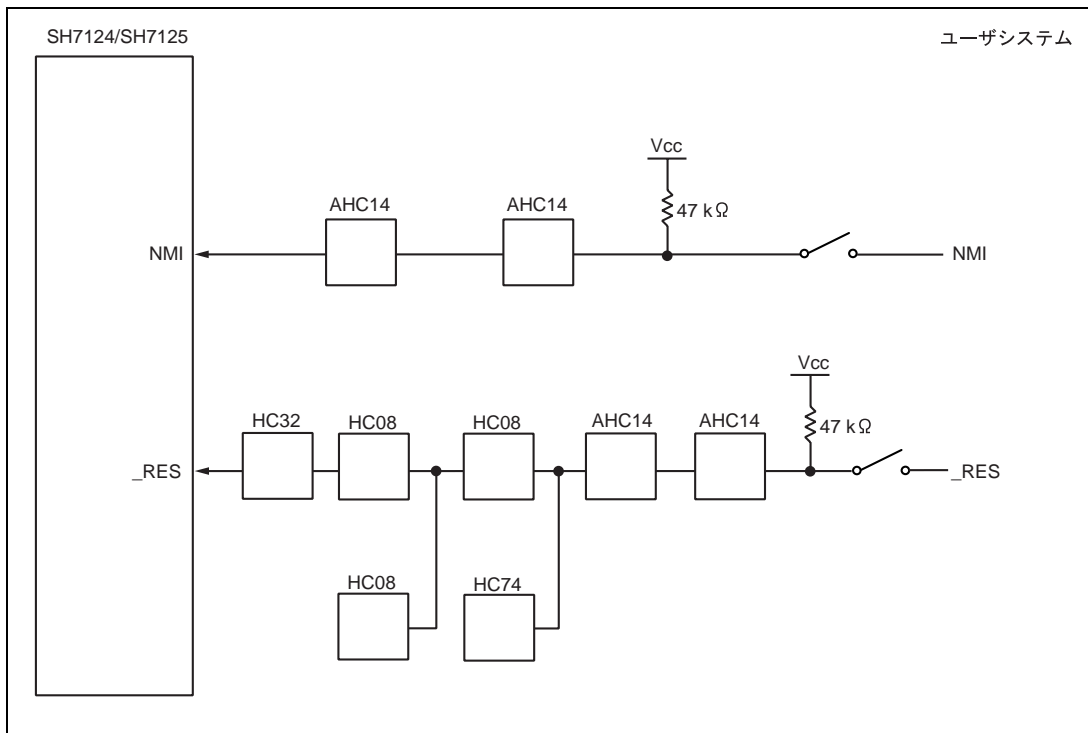
図 3.9 ユーザインタフェース回路(3)
