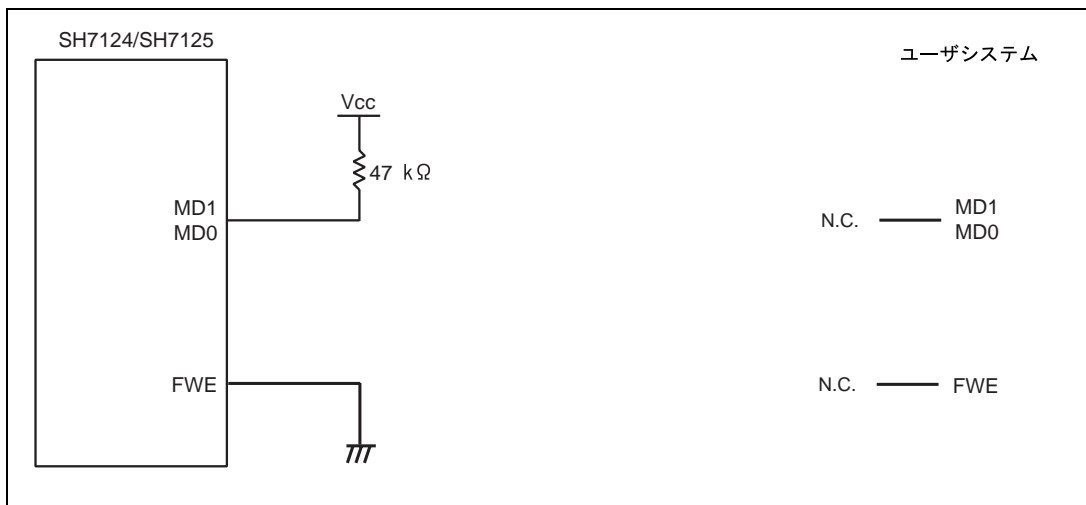
図 3.7 ユーザインタフェース回路(1)
