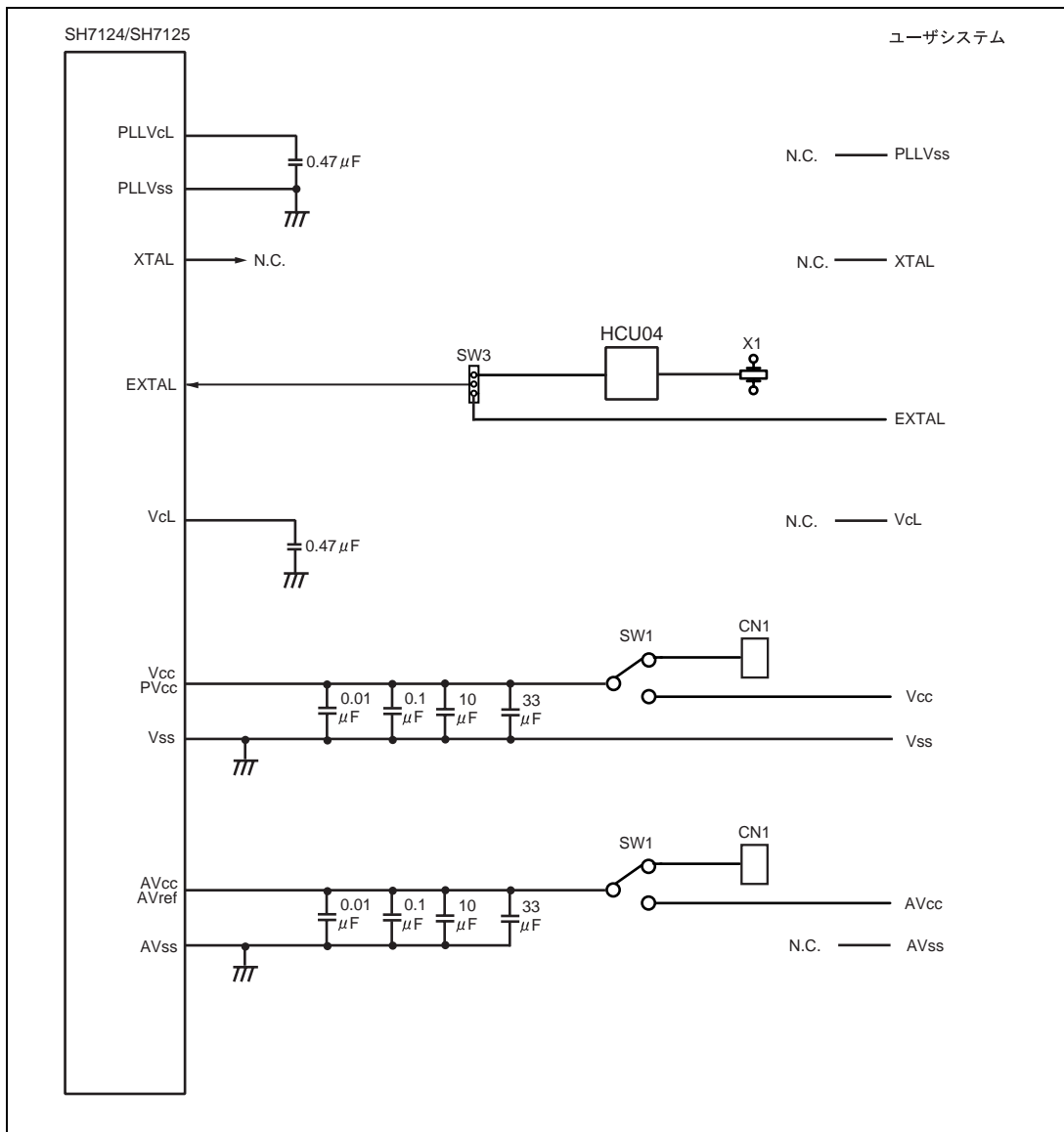
図 3.10 ユーザインタフェース回路(4)
