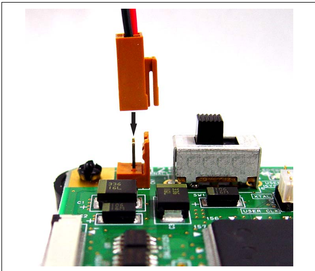
図 2.7 デバッグ MCU ボードと電源ケーブルの接続
