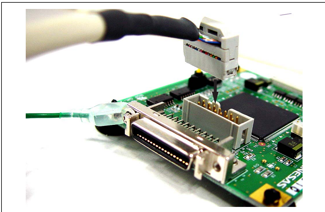
図 2.4 デバッグ MCU ボードとユーザインタフェースケーブル(14 ピン)の接続
