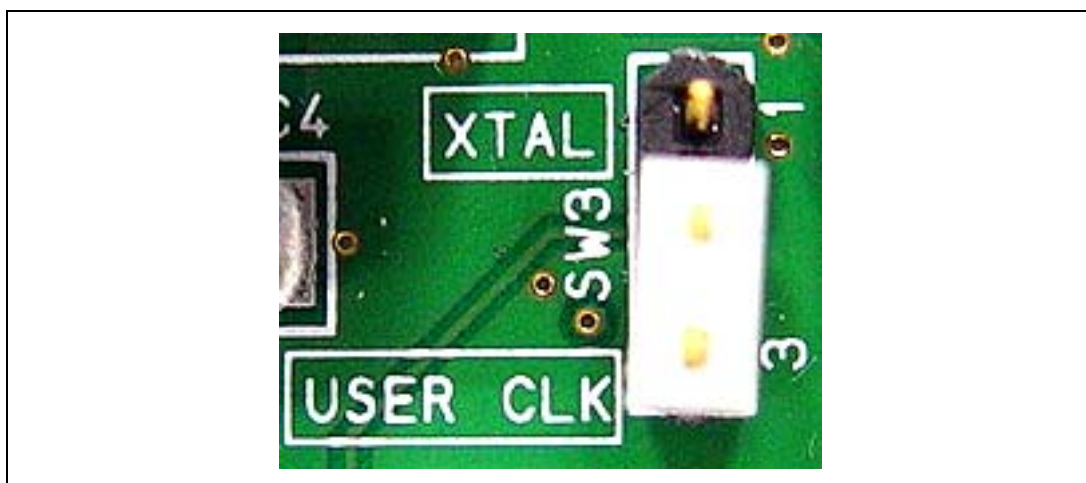
図 2.8 クロック選択ジャンパ
