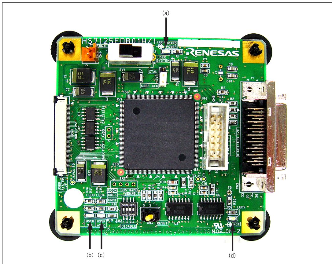
図 1.3 デバッグ MCU ボード本体の上面(1)
