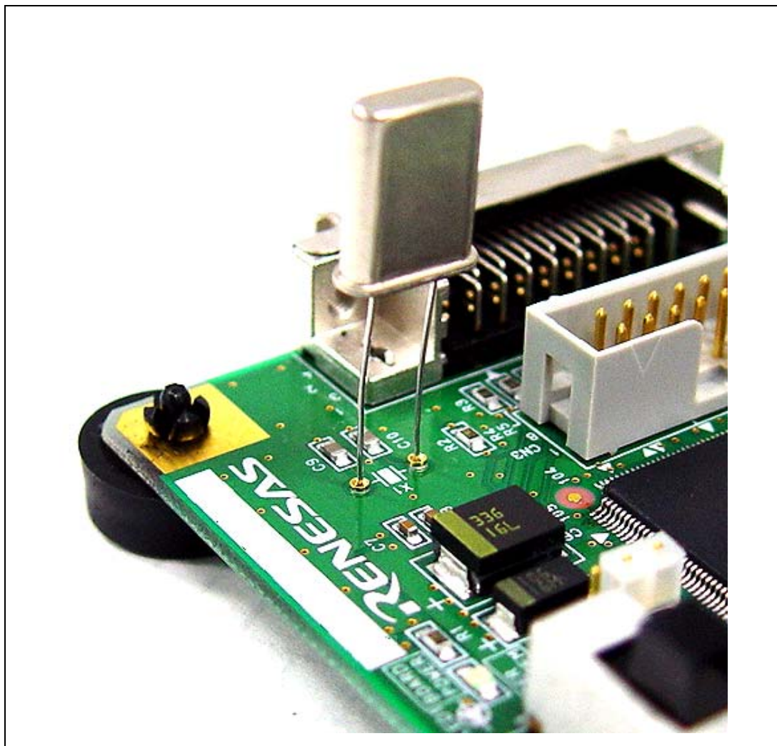
図 2.9 水晶発振子の実装
