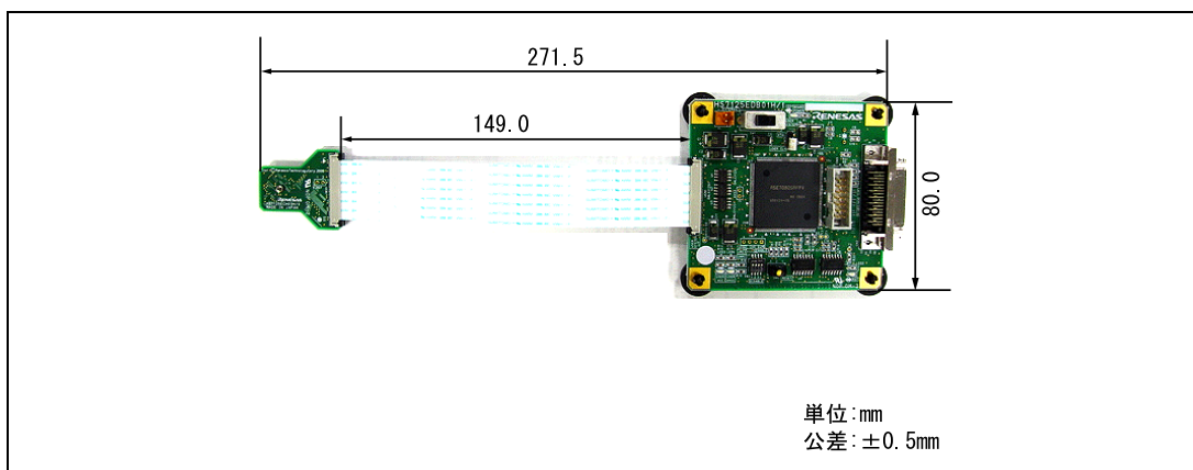
図 3.1 デバッグ MCU ボードの外形寸法図
