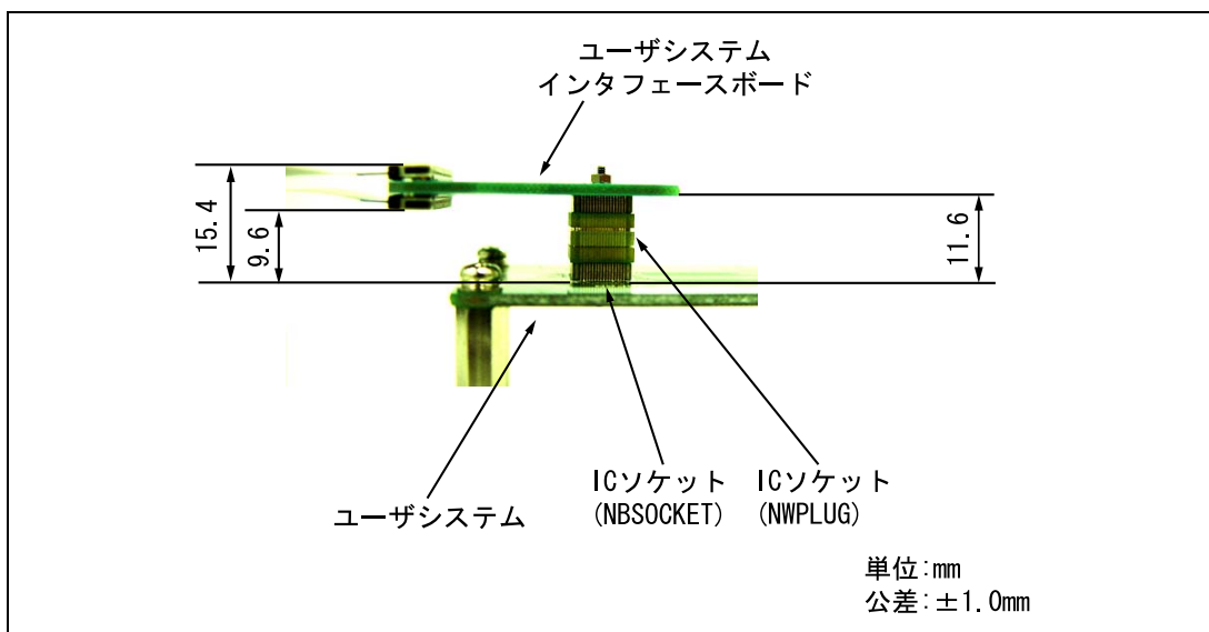
図 3.4 ユーザシステムインタフェースボード接続時のユーザシステムとの寸法
