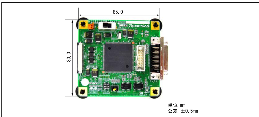
図 3.2 デバッグ MCU ボード本体の外形寸法図
