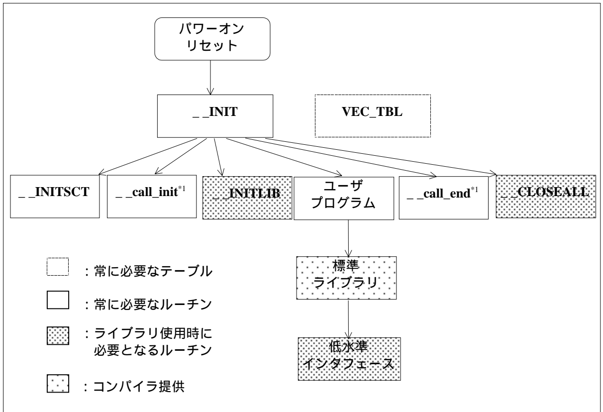
図 3-5 プログラムの構成例 (ライブラリ関数を使用する場合)
