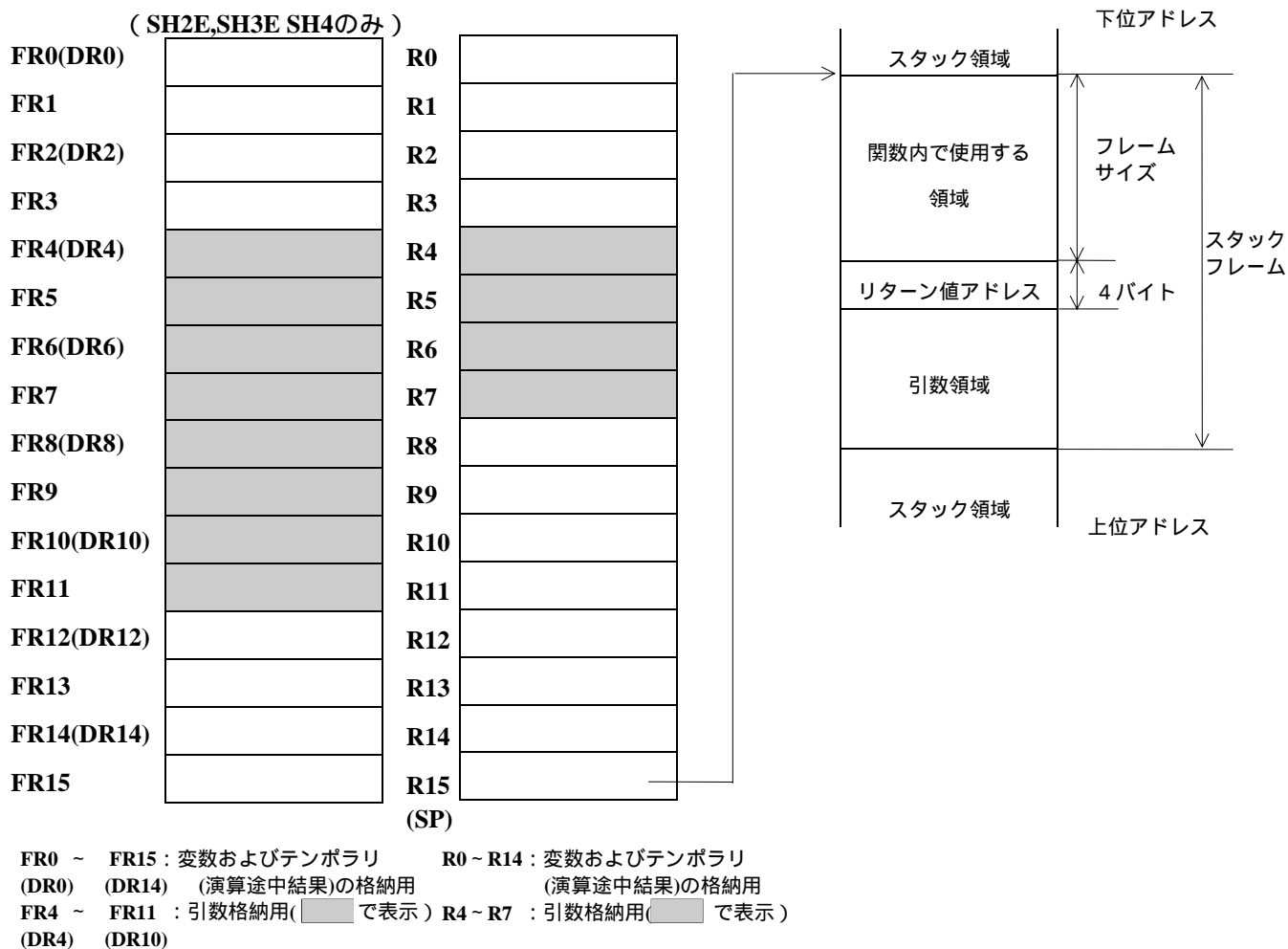
図 C-1 レジスタとスタック領域の使用法
