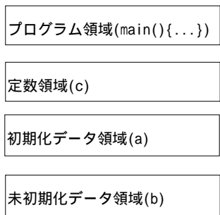
コンパイラが生成する領域と格納されるデータ
