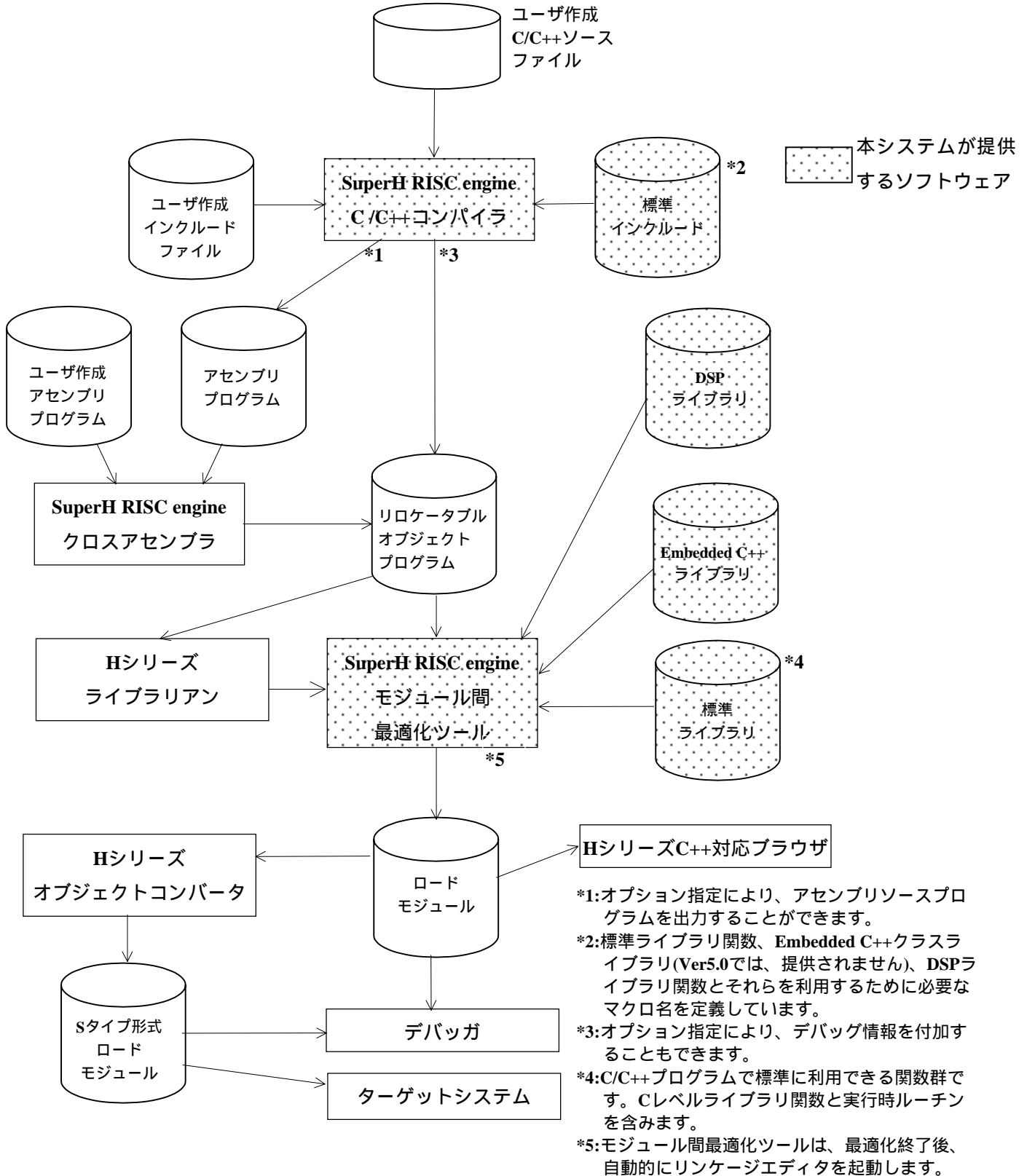
図 1-2 プログラムの開発手順
