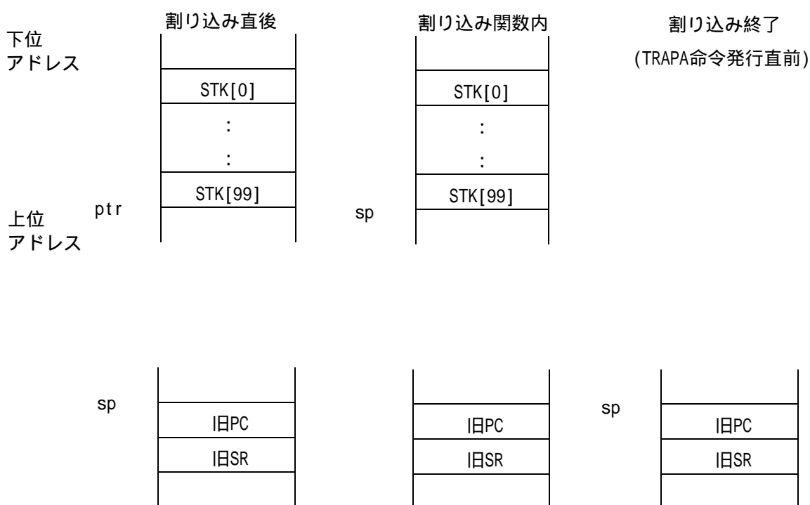
図 2-5 割り込み関数によるスタック使用例
