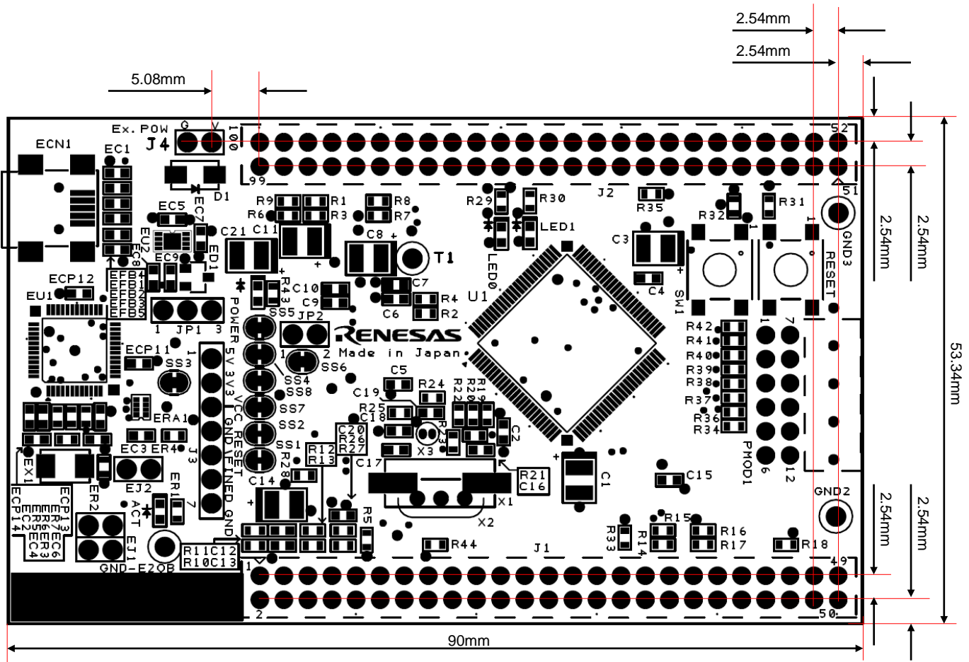
図 3-1：部品配置図
