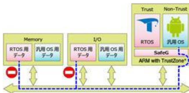
TOPPERS-Pro SafeG-Mブロック図
