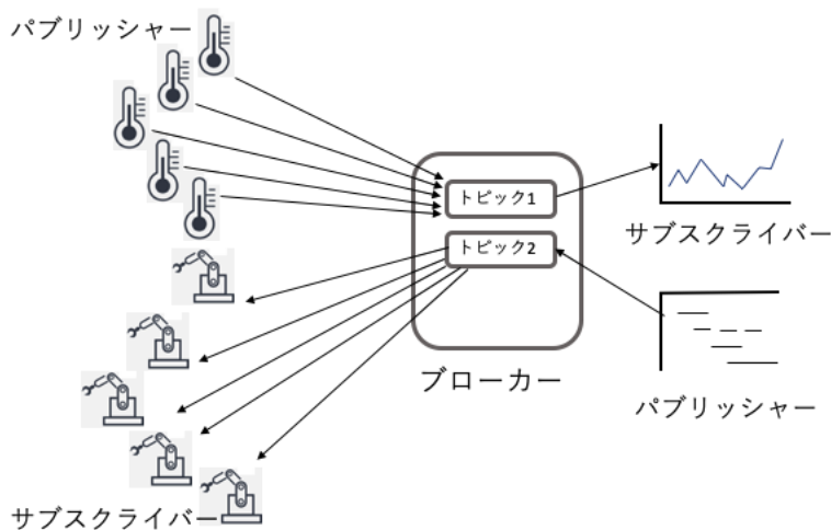
MQTTのパブリッシュ・サブスクライブ
