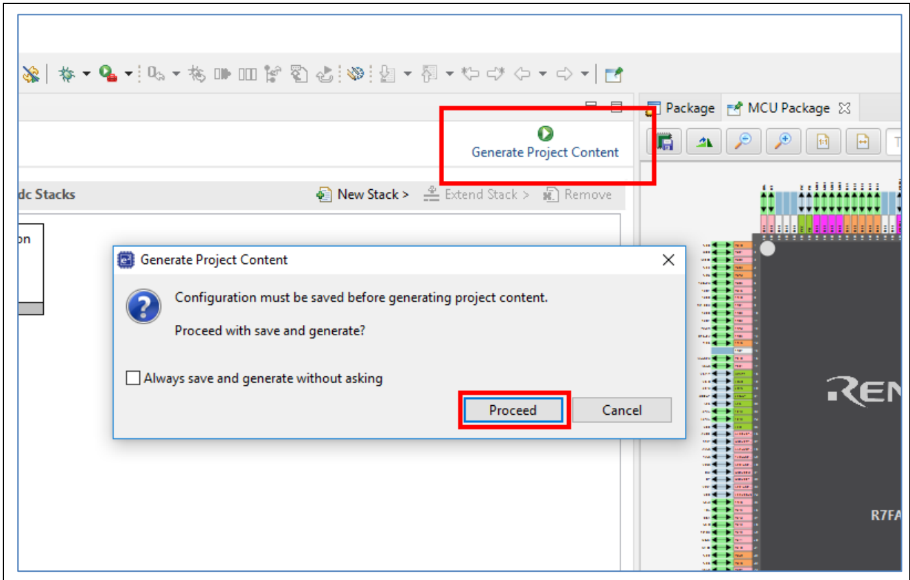
図 20. 設定変更の保存
