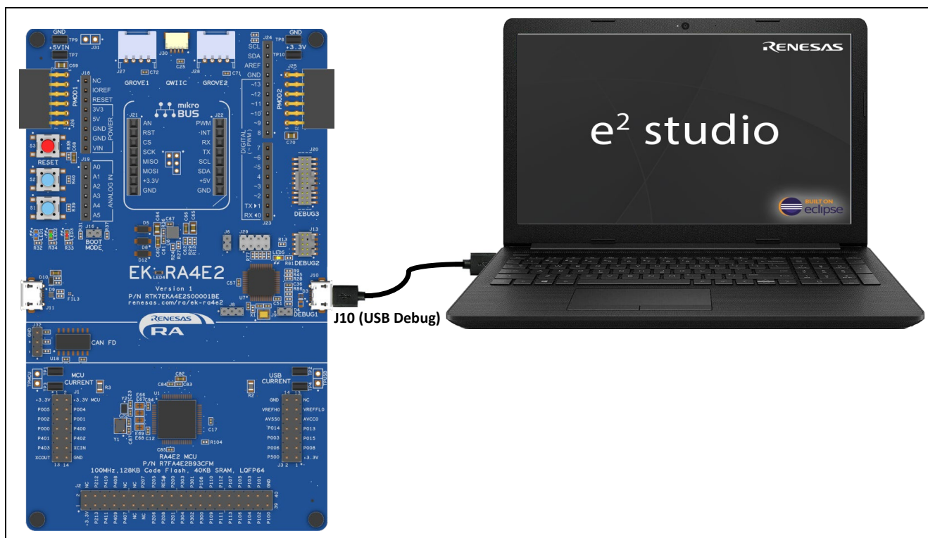
図 23. USB デバッグポートを使用した EK-RA4E2 ボードとホスト PC の接続
