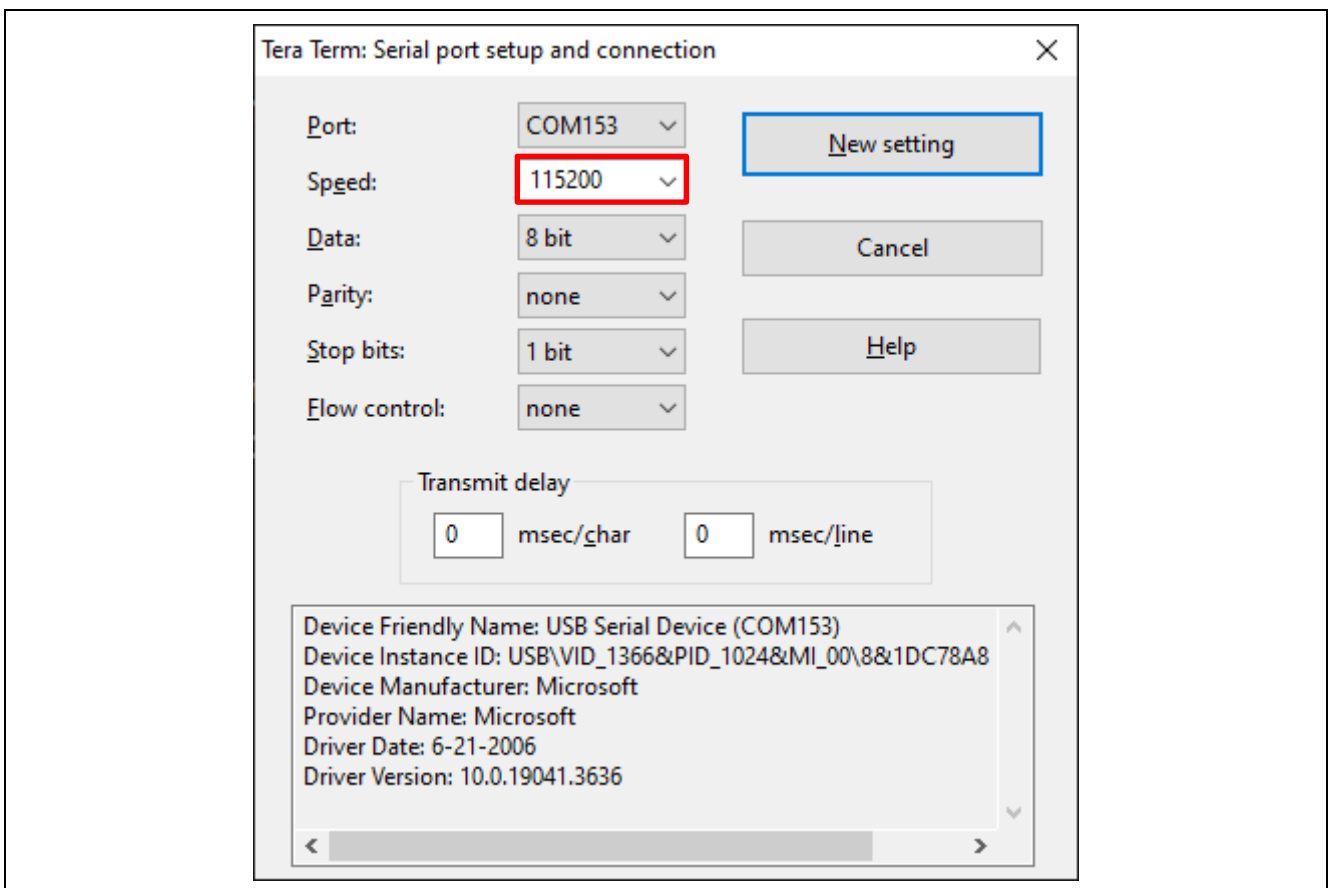
図 6. [Speed]プルダウンで 115200 を選択
