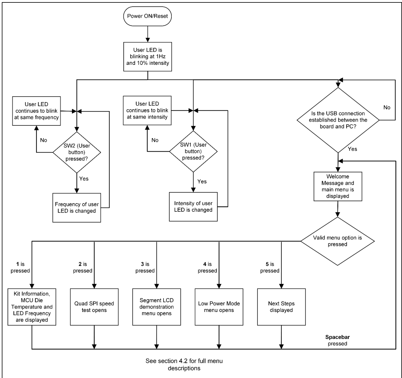
図 2. クイック スタート サンプル プロジェクトフロー
