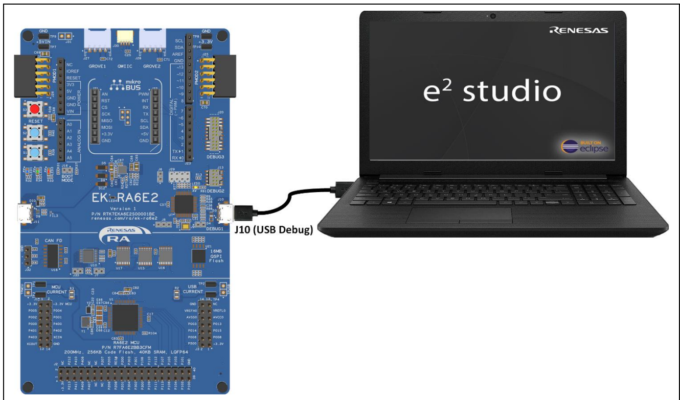
図 23. USB デバッグポートを使用した EK-RA6E2 ボードとホスト PC の接続
