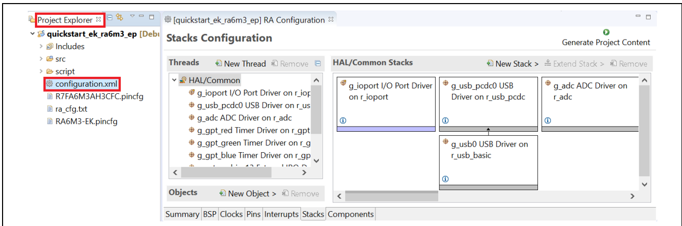
図 16 コンフィグレータの起動
