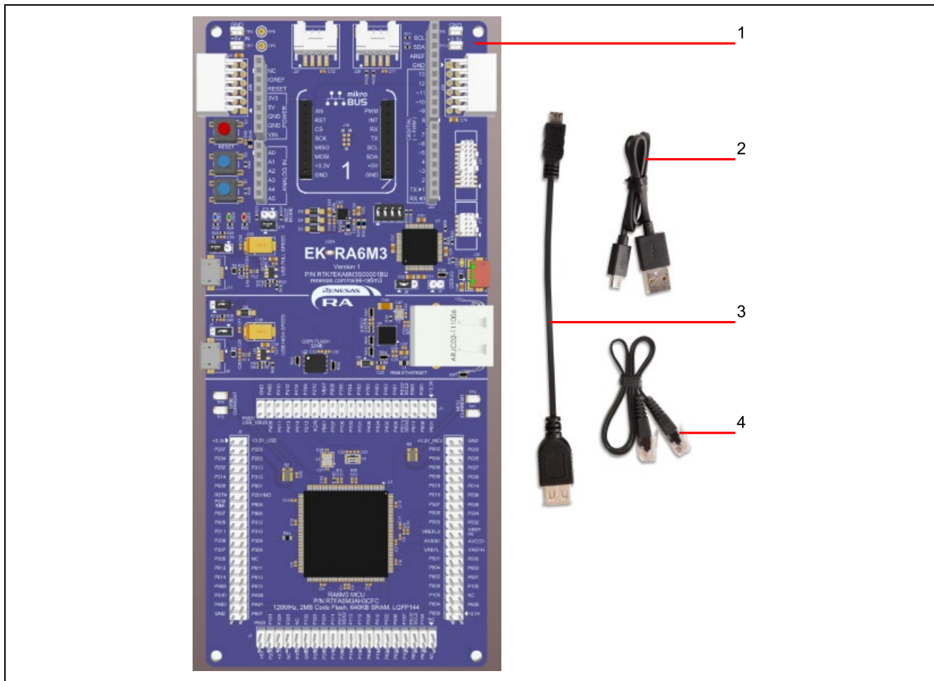
図 1 EK-RA6M3 評価キット構成
