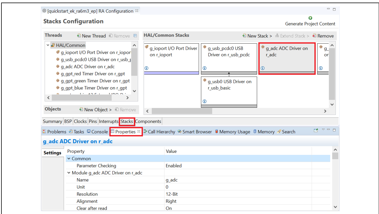
図 17 構成設定の修正
