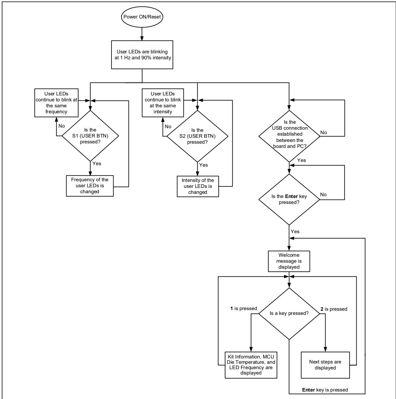
図 2 クイックスタートサンプルプロジェクトのフロー
