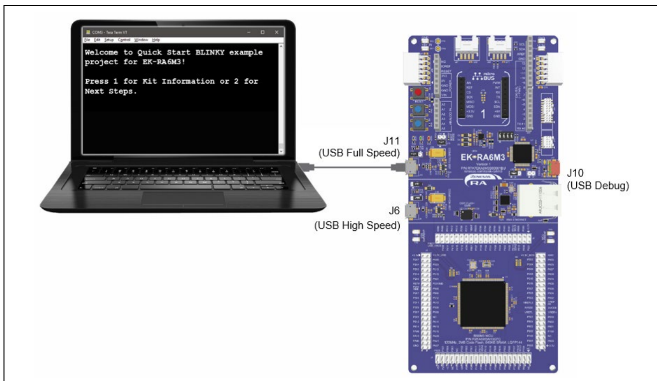
図 3 EK-RA6M3 ボードを USB フルスピードポートからホスト PC に接続
