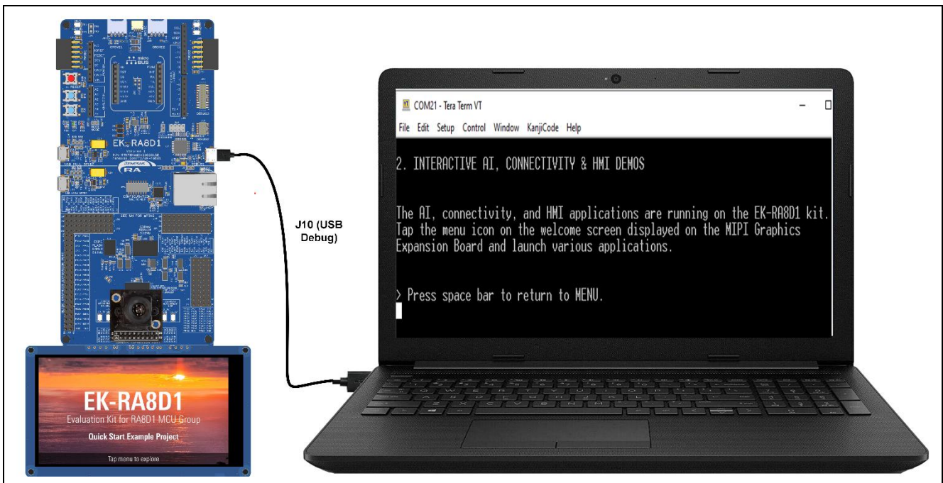
図 7. EK-RA8D1 ボードを USB フルスピードポート経由でホスト PC に接続
