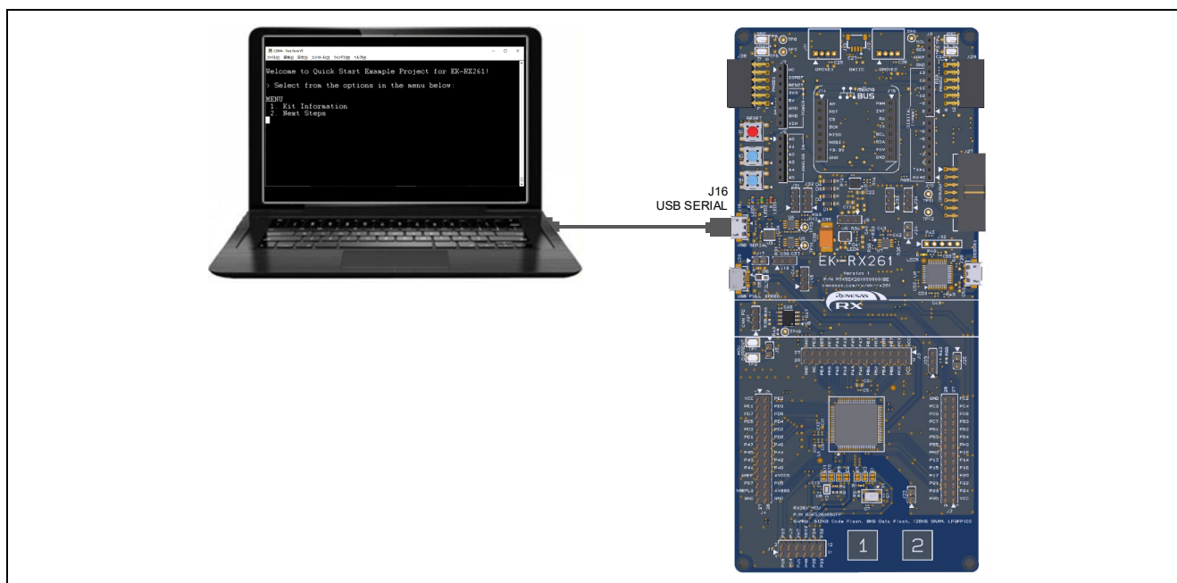
図 3 EK-RX261 を USB コネクタ（J16）経由でホスト PC に接続
