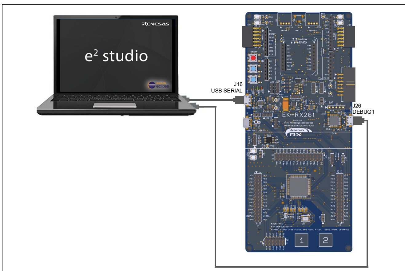
図 23 USB デバッグポートを介して EK-RX261 をホスト PC に接続
