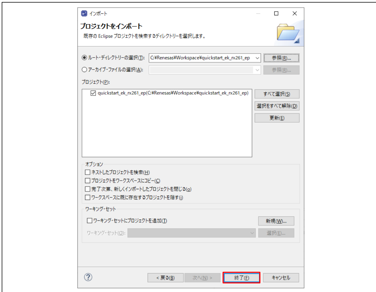
図 16 Quick Start Example Project のインポートを完了する
