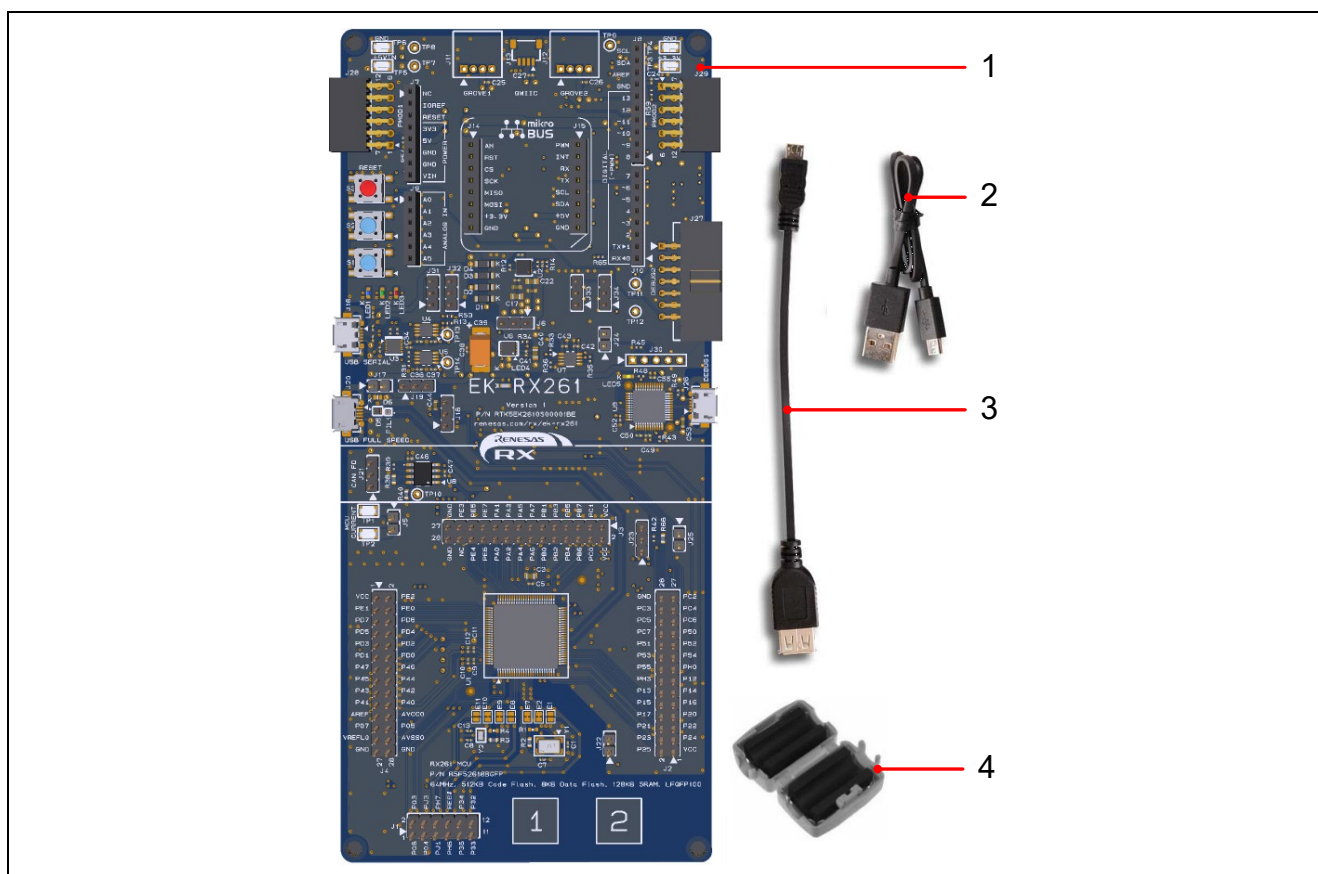
図 1 EK-RX261 評価キット構成
