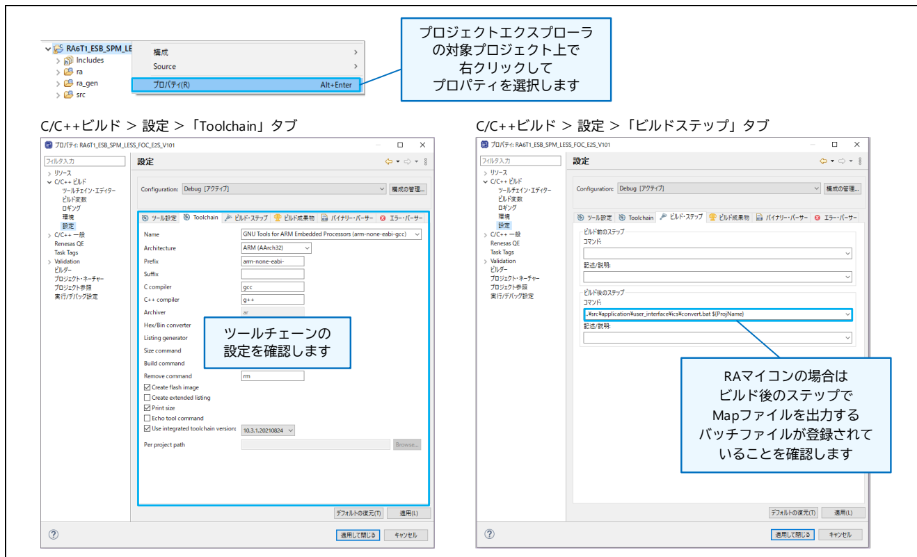
図 2-12 ツールチェーンの設定
