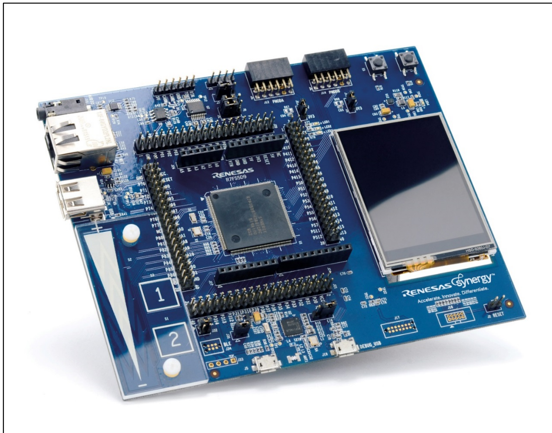
図 1 PK-S5D9 メインボード
