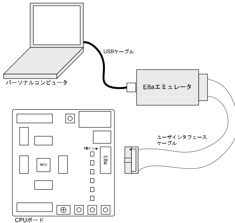
図 5-2: 接続例
