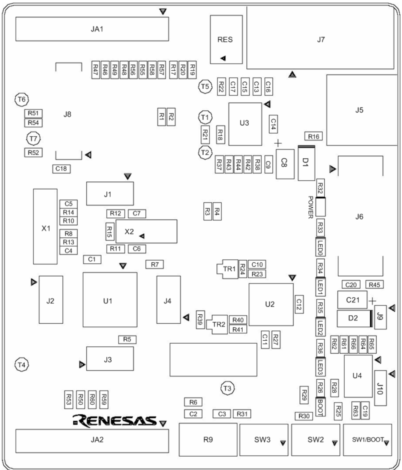
图 11-1: 部品配置図
