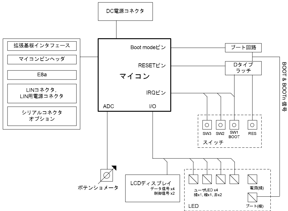
図 5-1: ブロック図
