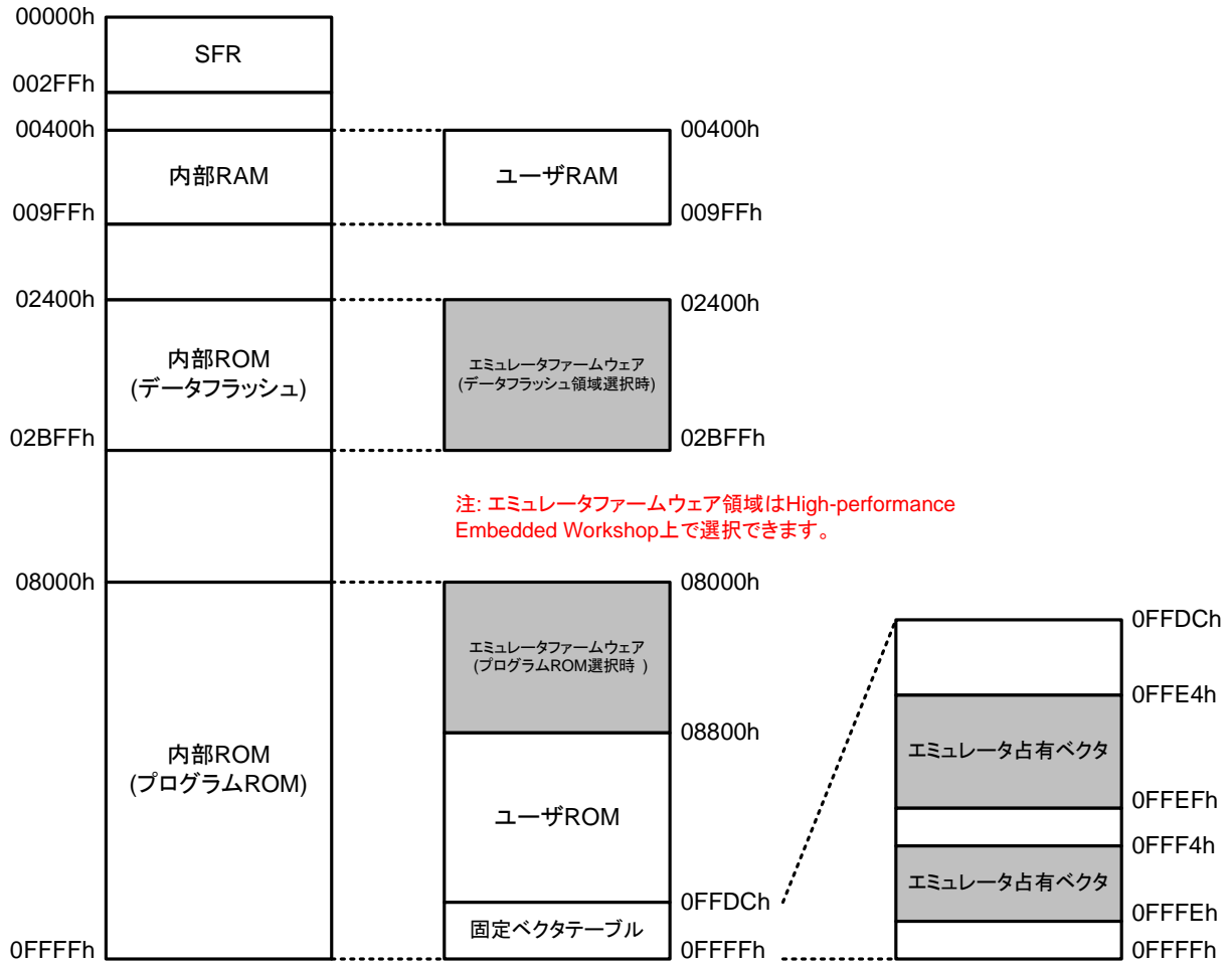
図 10-1: メモリマップ
