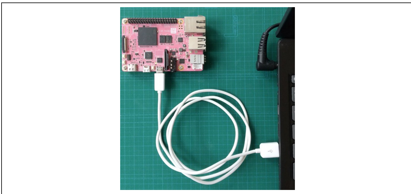
図 6-4 ターゲットボードと PC の接続
