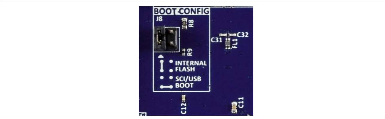
図 2 ボード起動時に動作モードを設定するジャンパー J8 の配置場所
