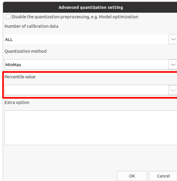
図 3-1 量子化詳細設定画面
