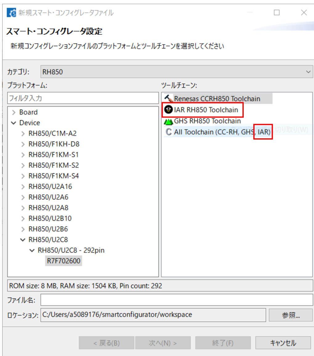
図 5-4 ツールチェーンの選択
