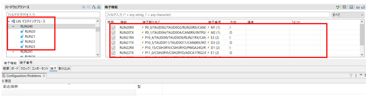
図 3-2 LIN マスタインターフェースの端子設定(修正後)
