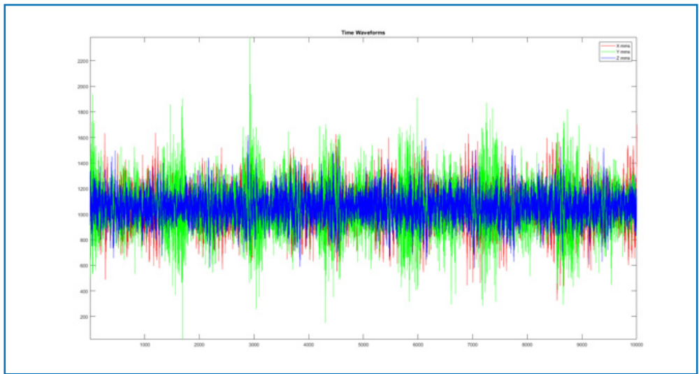
Figure 8 – 加速度計から直接サンプリングされた生の時間波形データ。このデータは情報密度が高いです。Figure 6 の単純平均とFigure 7のFFTの両方を計算した生データです。ここでは、トランジェントや位相などの重要なタイム情報とともに、非常に詳細な周波数情報が得られます。しかし、ノイズも多くあります。そのため、このようなデータを人間のアナリストが直接使用することは非常に困難です。しかし、Reality AIのようなデータドリブンな特徴検出アルゴリズムでは、この種のデータから最大値を抽出して、まさにその信号の部分に焦点を絞リカスタムの変換を作成します。検出問題に関連する信号の部分だけを、です。
