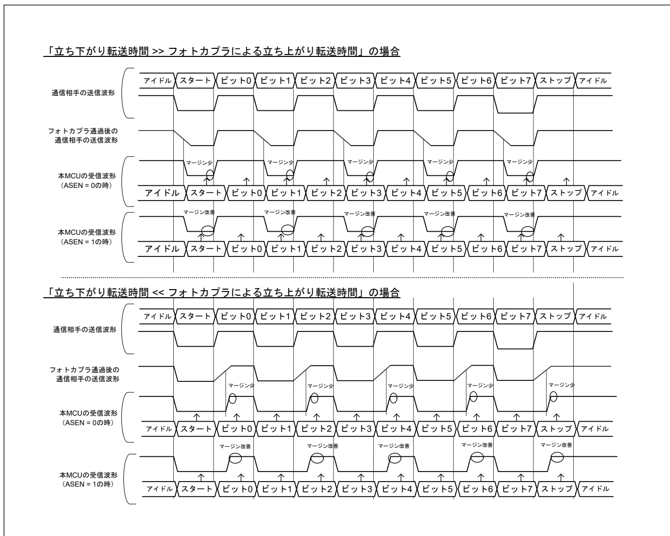
図 29.33 受信サンプリングタイミング調整機能による受信マージン向上の例
