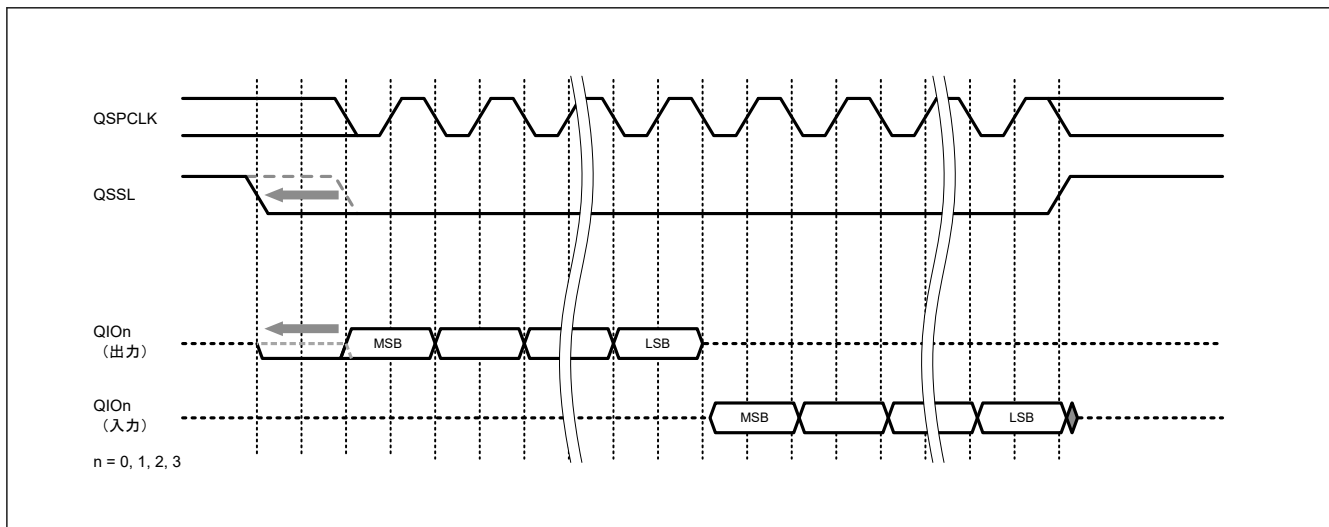
図 33.11 SFMSLD ビットを使用した QSSL 信号のセットアップ時間調整
