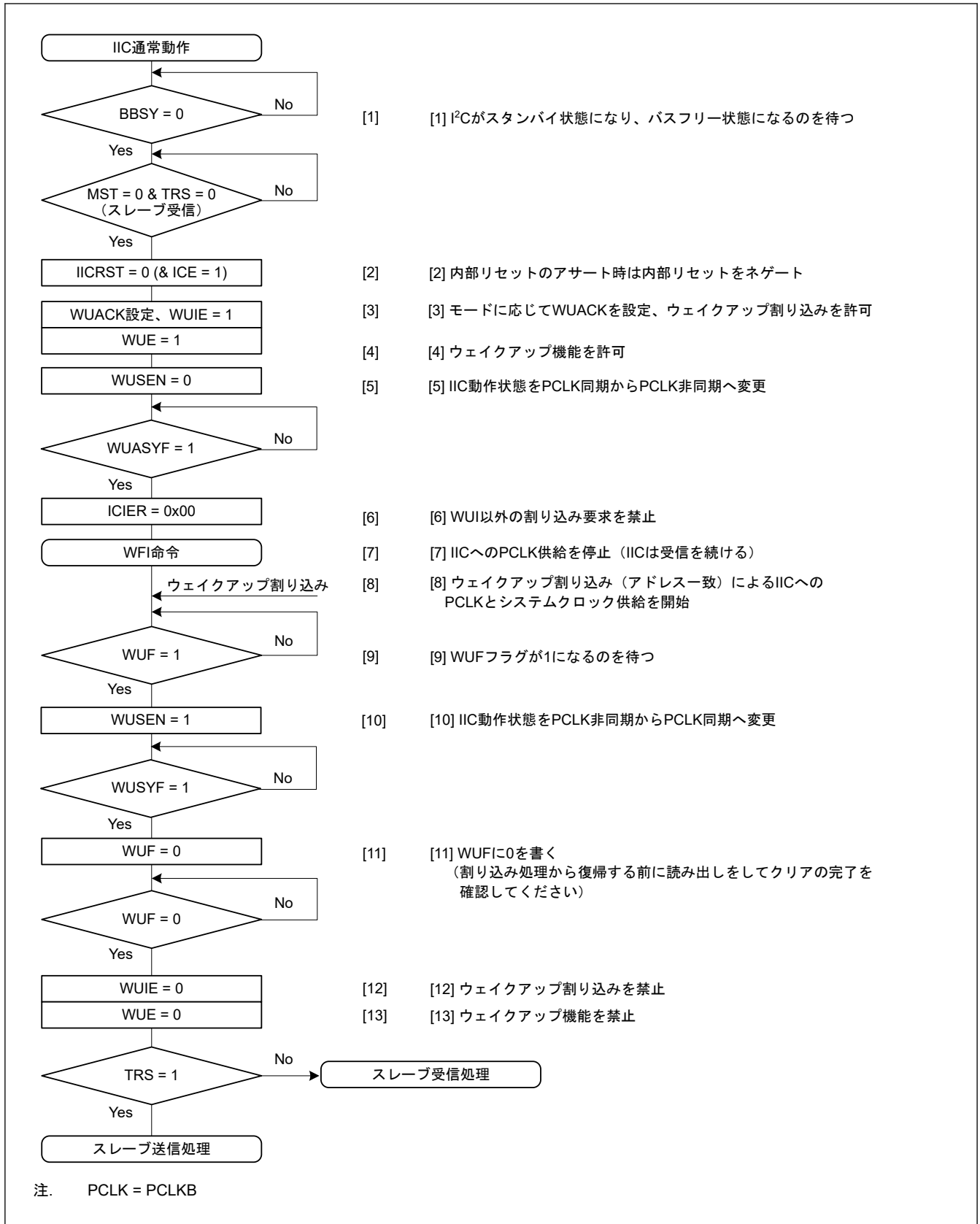
図 30.33 ノーマルウェイクアップモード2の動作例 (スレーブアドレス一致時のウェイクアップ割り込みによるウェイクアップの場合)
