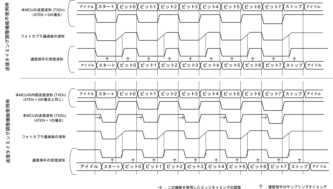
図 29.37 フォトカブラを経由する送信波形の説明
