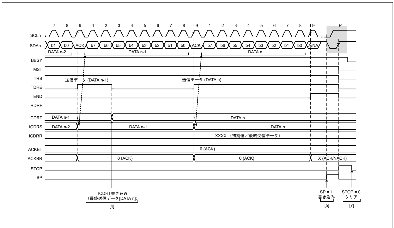
図 30.9 マスタ送信の動作タイミング (3)
