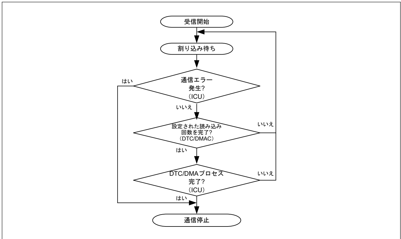
図 34.55 受信手順
