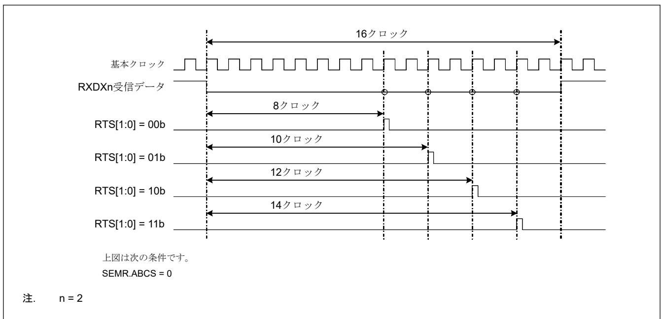
図 29.114 RXDXn 受信データサンプリングタイミング
