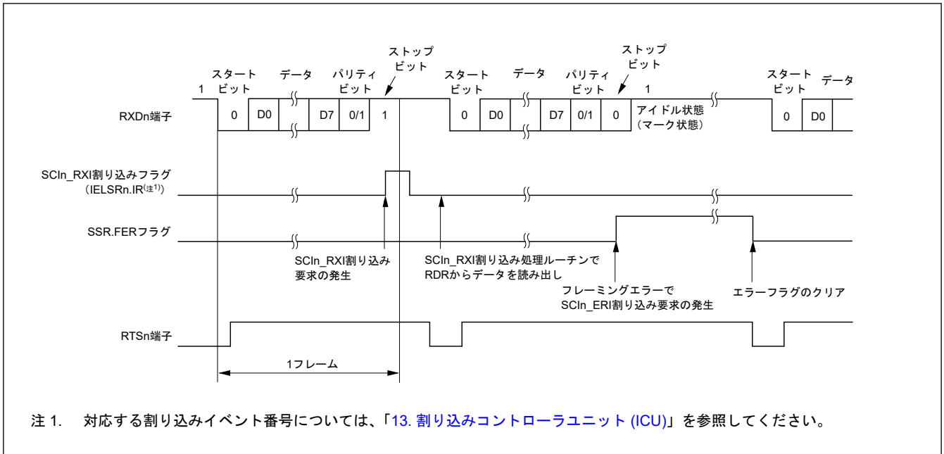
図 29.19 調歩同期式モードにおけるシリアル受信の動作例 (2) (RTS 機能を使用する場合) (8 ビットデータ/パリティあり/1 ストップビットの場合)
