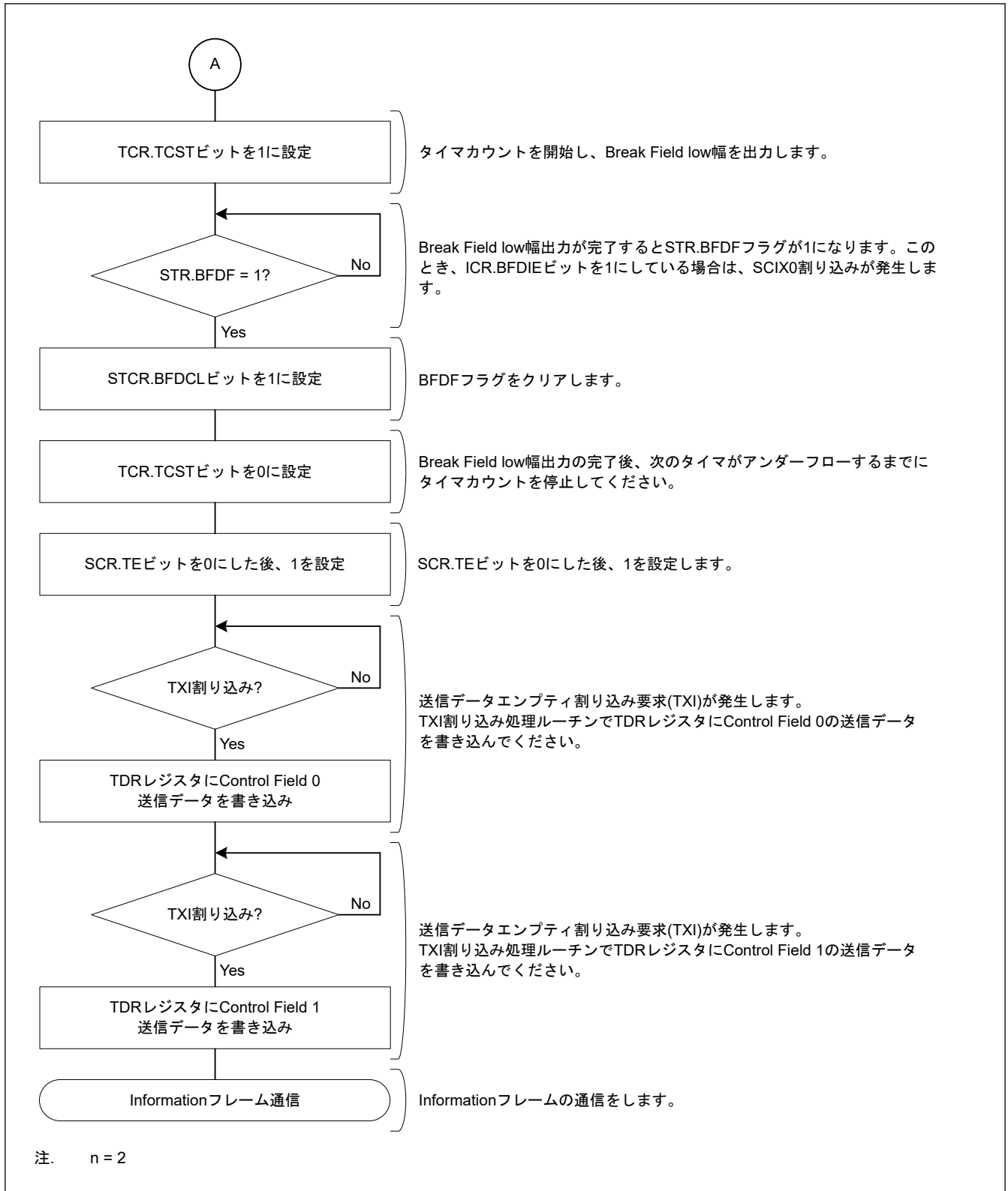
図 29.104 Start Frame 送信フローチャート例 (2/2)
