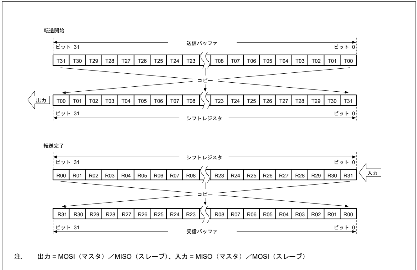
図 32.16 LSB ファースト転送 (32 ビットデータ/パリティ機能無効)
