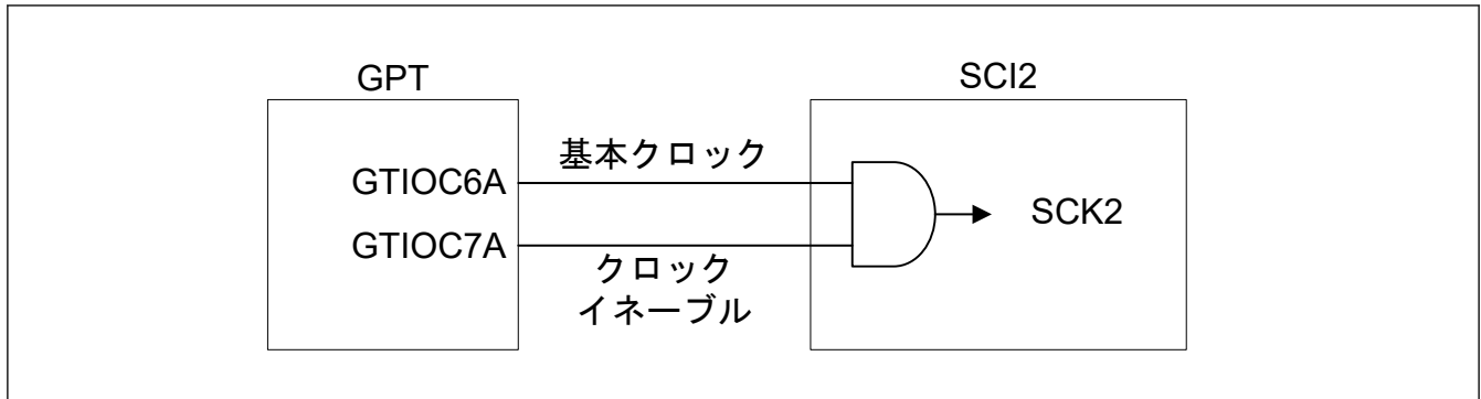
図 29.3 GPT と SCI の接続例
