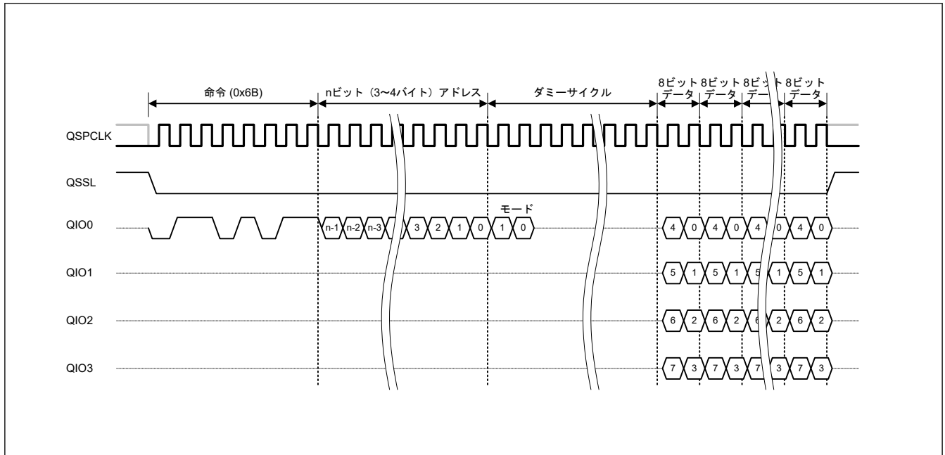
図 33.25 拡張 SPI プロトコルでのファストリード Quad 出力バスサイクル
