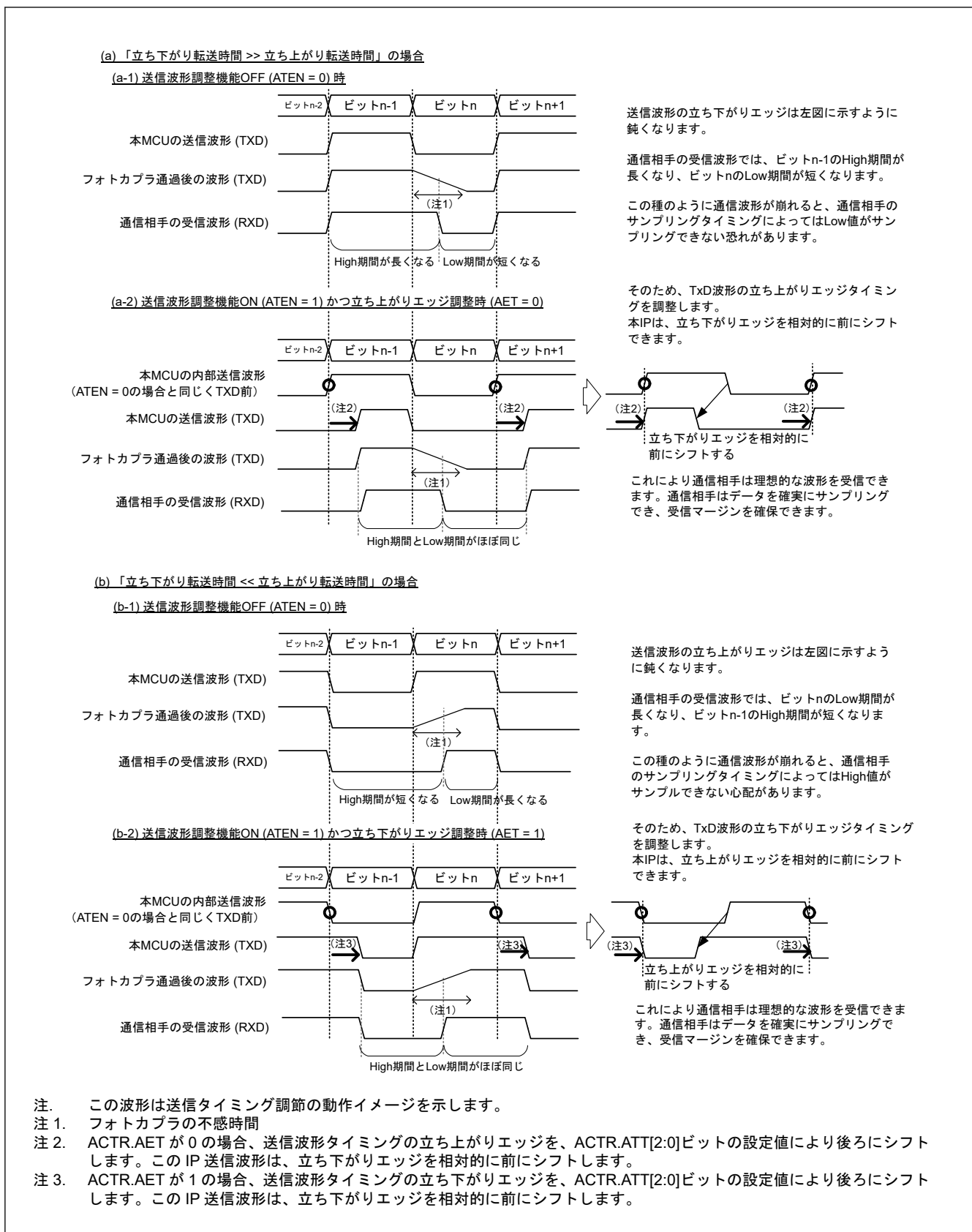
図 29.36 フォトカプラを通過する通信の送信動作の概要
