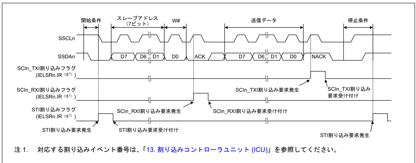
図 29.94 簡易 IIC モードにおけるマスタ送信の動作例 2 (7 ビットスレーブアドレス、ACK 割り込み、NACK 割り込み使用時)
