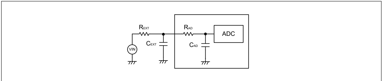
図 39.35 サンプル&ホールド回路の簡略図
