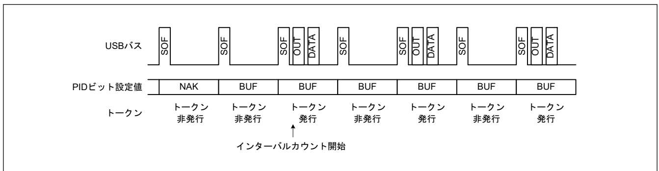
図 28.18 IITV[2:0] = 1 の場合のトークン発行の有無
