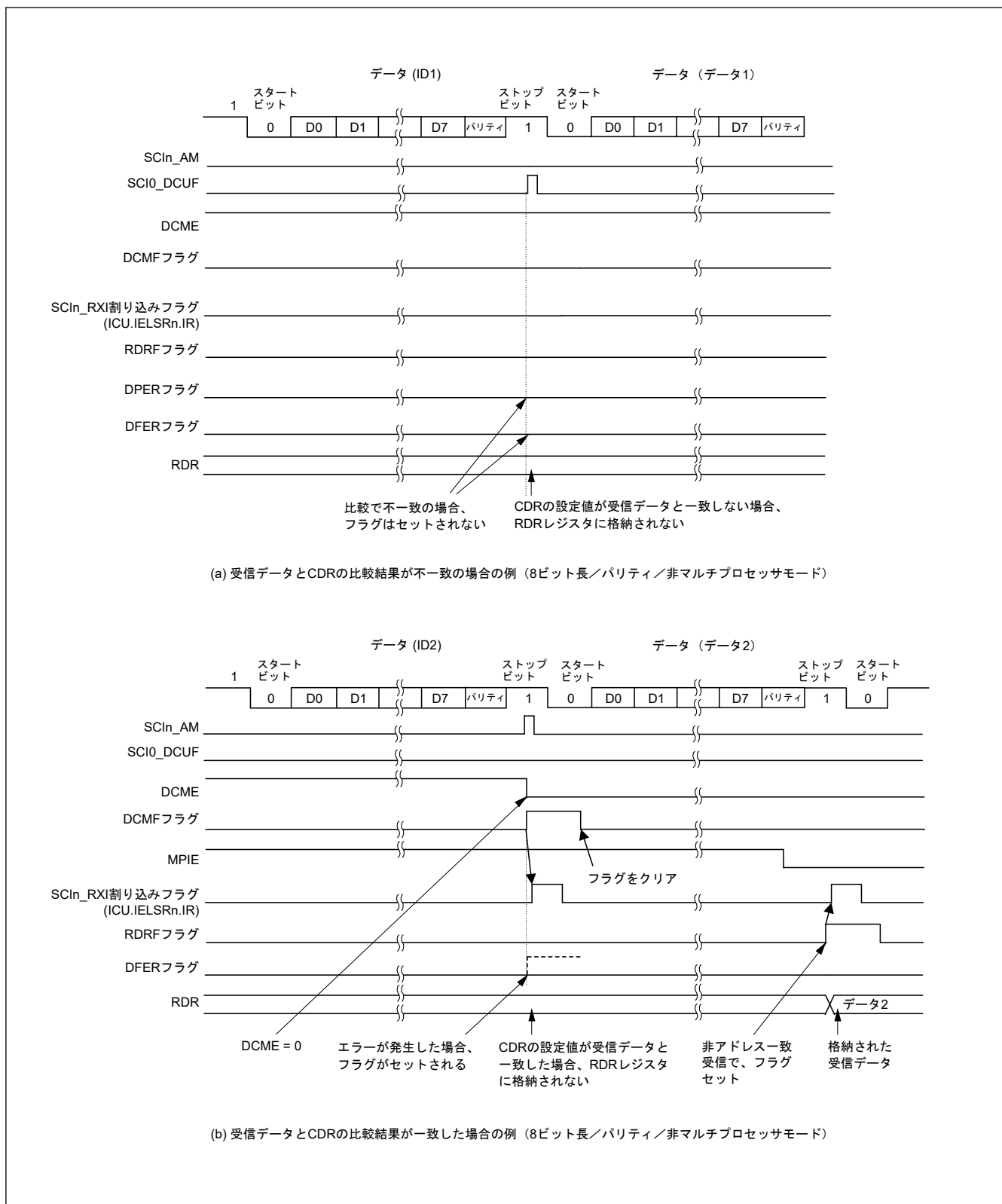
図 29.9 アドレス一致検出の例 (1) (通常モード)
