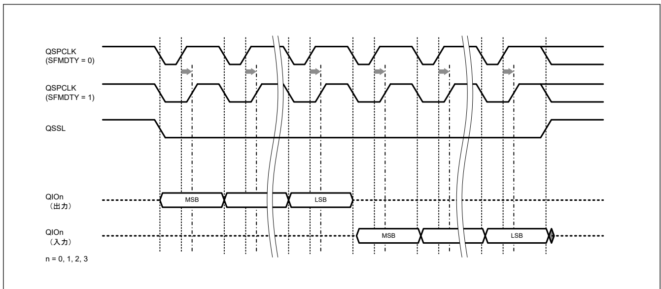
図 33.10 PCLKA を 3 通り倍した場合の SFMDTY ビットを使用した QSPCLK 信号デューティー比補正例
