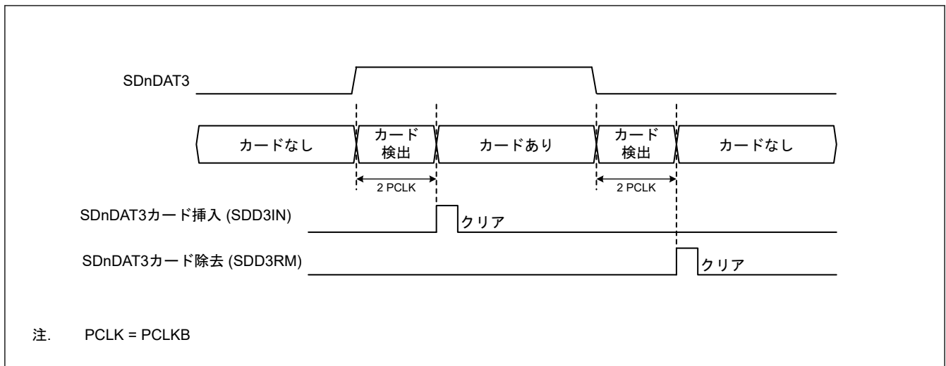
図 35.7 SDnDAT3 による SD カード検出
