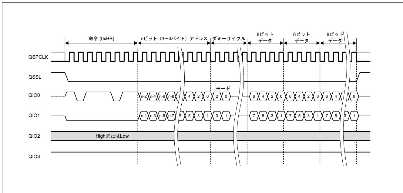
図 33.23 ファストリード Dual I/O バスサイクル(拡張 SPI プロトコル時)
