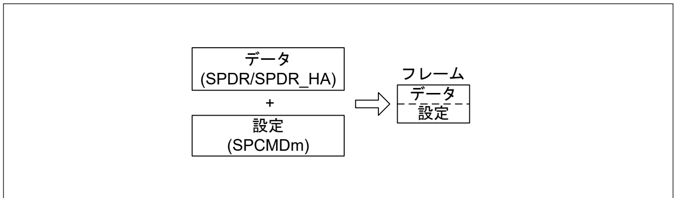
図 32.44 フレームの概念図
