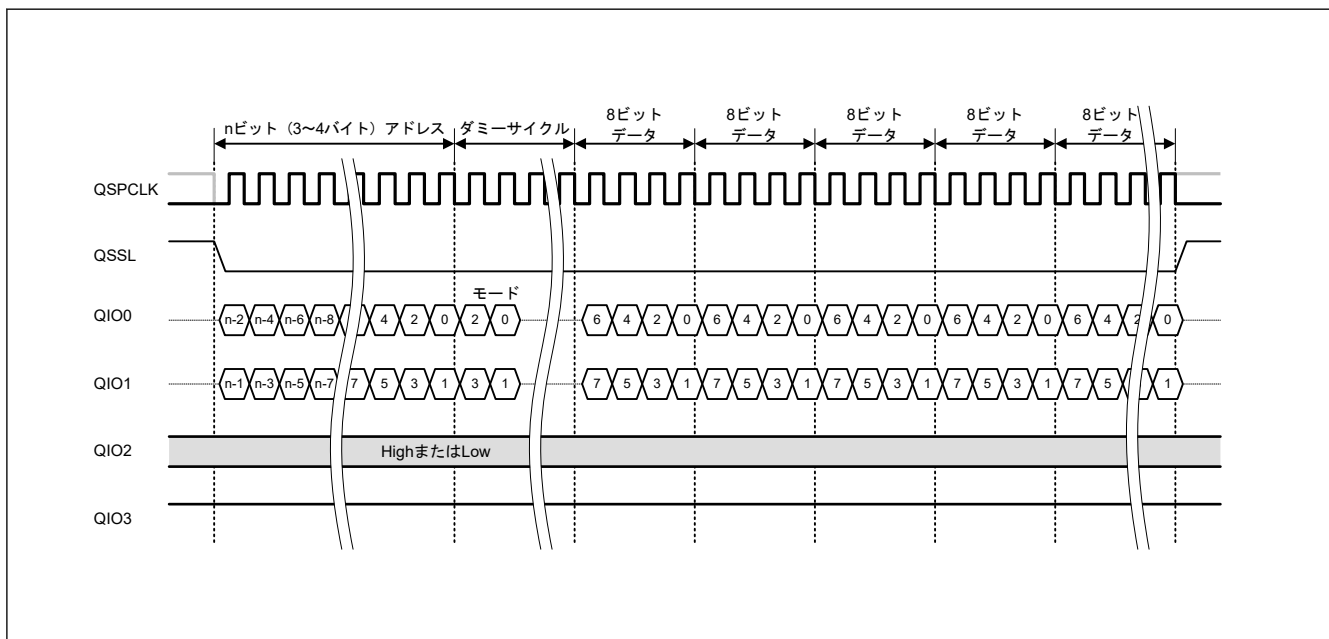
図 33.24 XIP モード時のファストリード Dual I/O バスサイクル
