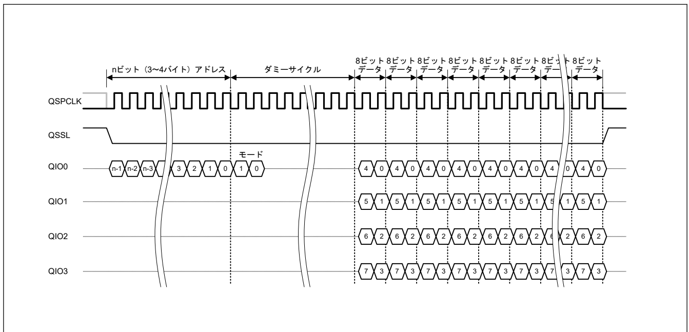
図 33.26 拡張 SPI プロトコルでの XIP モードファストリード Quad 出力バスサイクル
