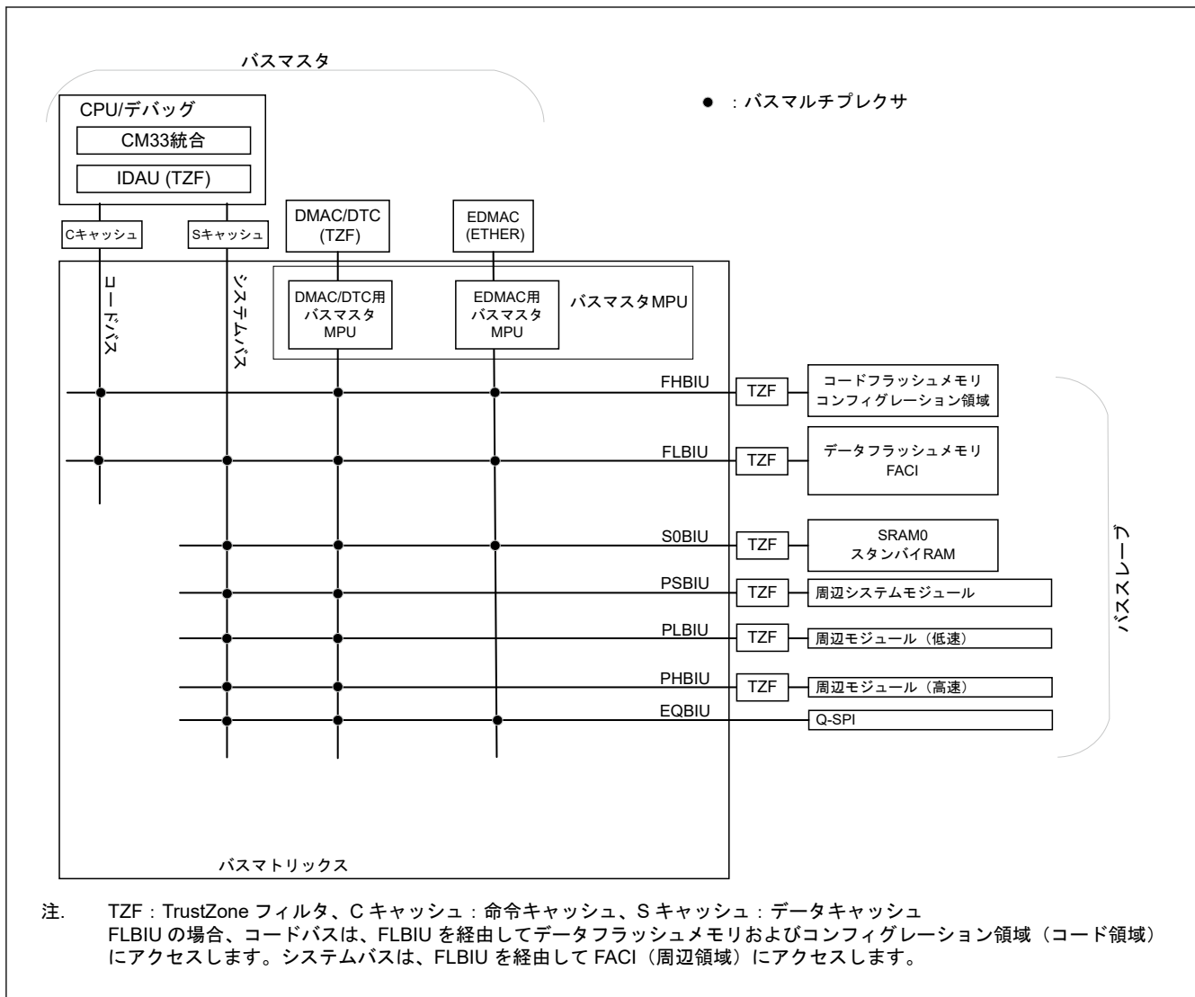
図 14.1 バス接続
