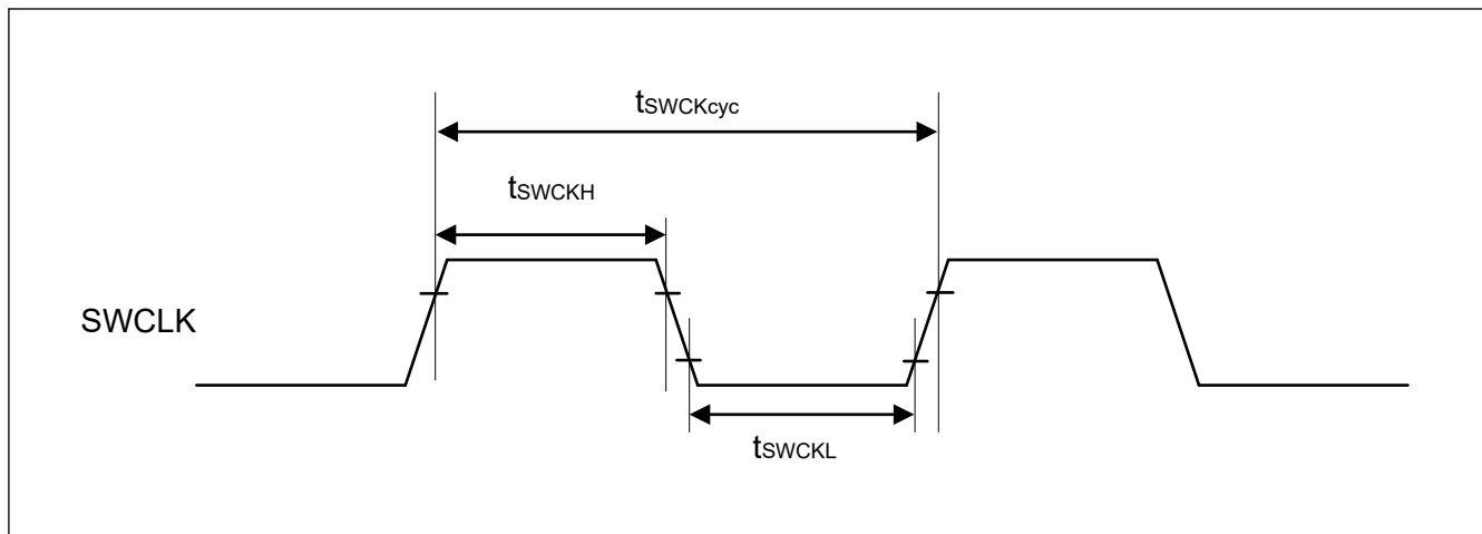
図 47.72 SWD SWCLK タイミング
