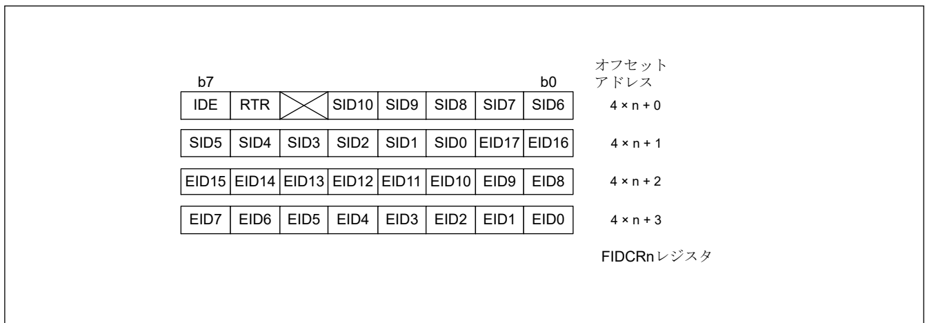
図 31.15 FIDCRn レジスタの構成 (n = 0)
