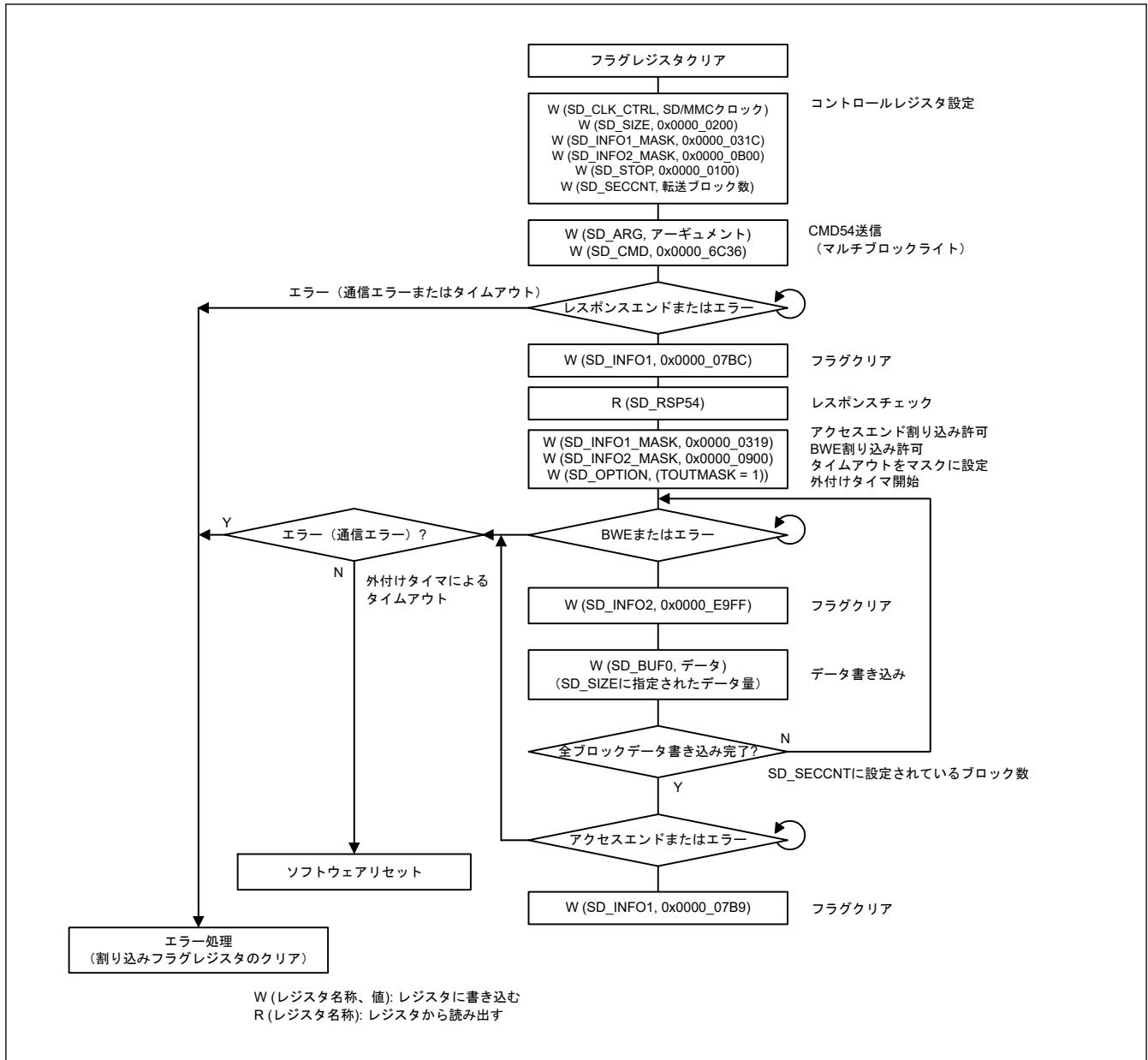
図 35.14 外付けタイマによるマルチブロックライト動作の例
