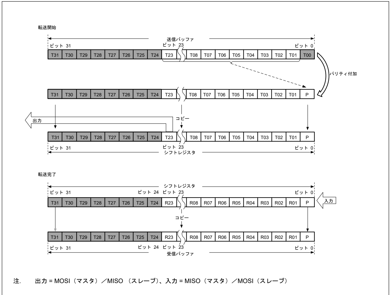
図 32.19 MSB ファースト転送 (24 ビットデータ/パリティ機能有効)
