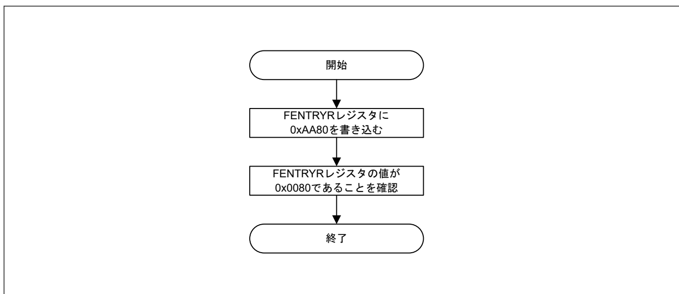
図 44.11 データフラッシュ P/E モードへの遷移手順
