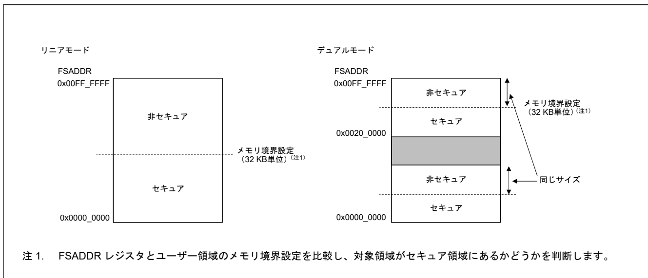
図 44.36 ユーザー領域のセキュア/非セキュア領域
