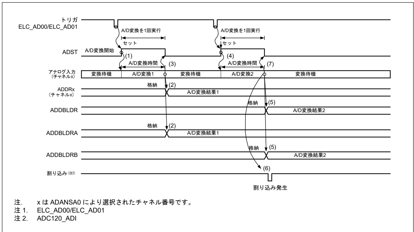
図 39.11 アナログ入力（チャンネル x）と ELC_AD00/ELC_AD01 の重複選択時のダブルトリガモード拡張動作例
