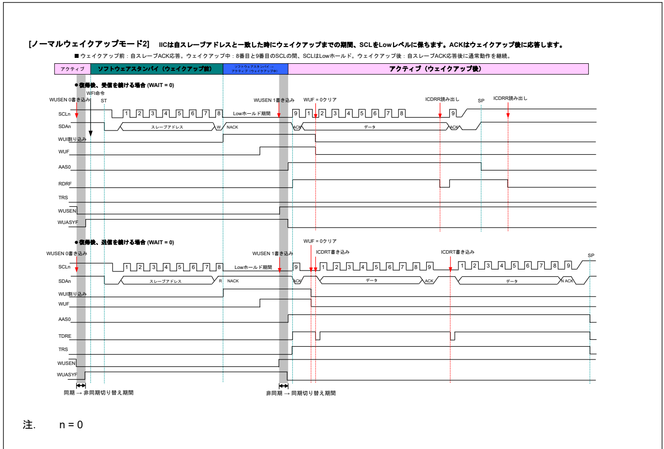
図 30.34 ノーマルウェイクアップモード2のタイミング
