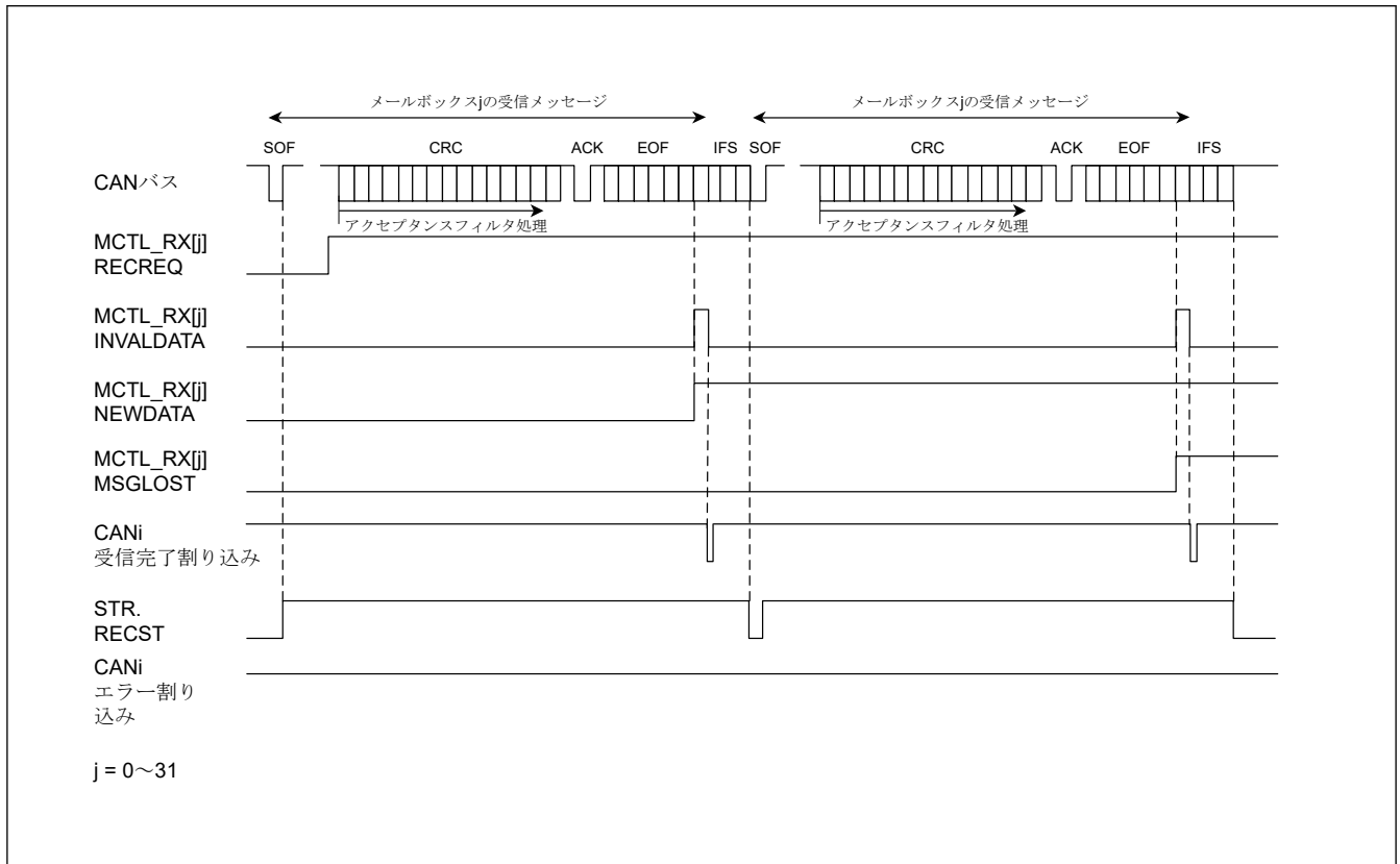
図 31.18 オーバーライトモードでのデータフレーム受信の動作例
