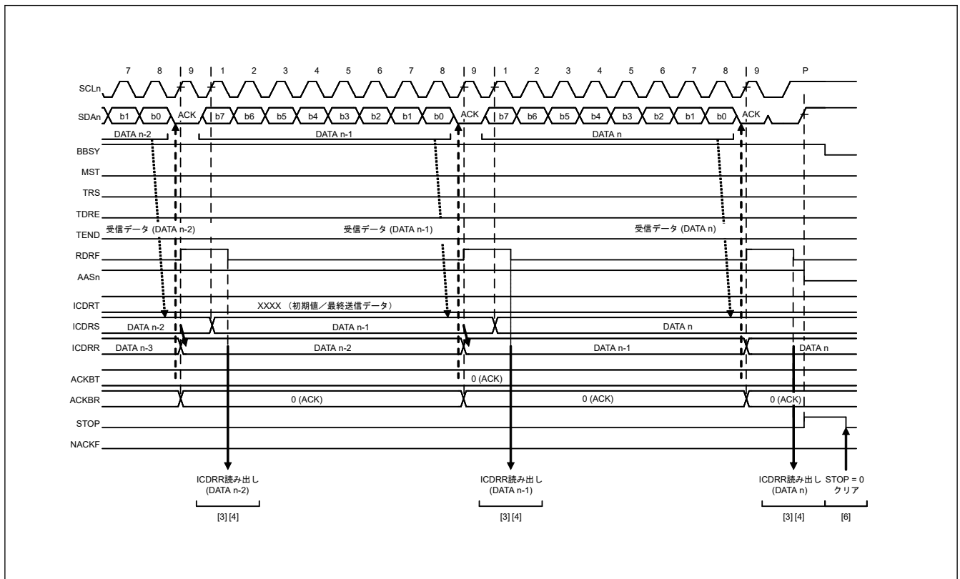
図 30.20 スleep受信の動作タイミング (2) (RDRFS = 0 の場合)
