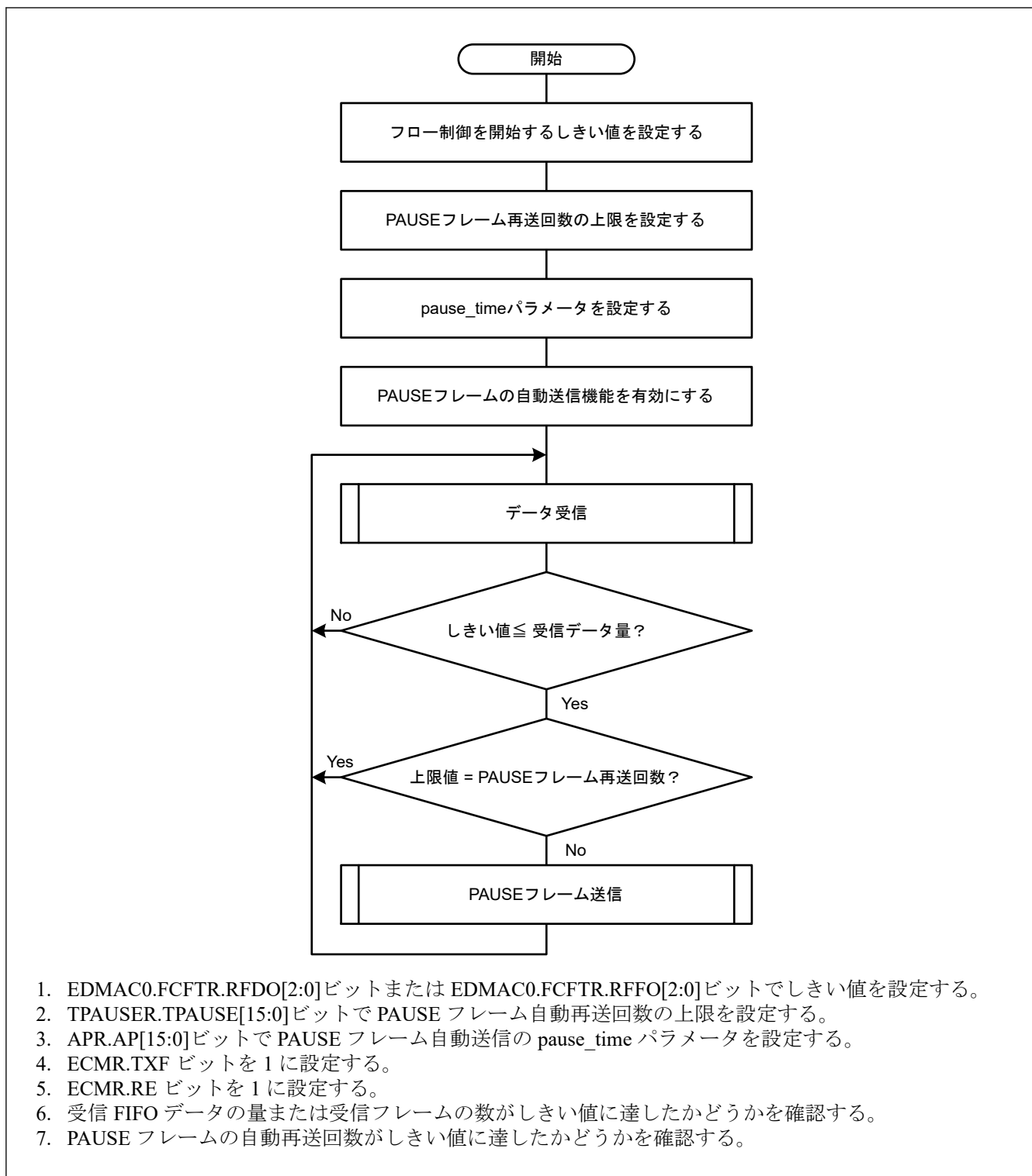
図 26.13 PAUSE フレーム自動送信の設定手順例
