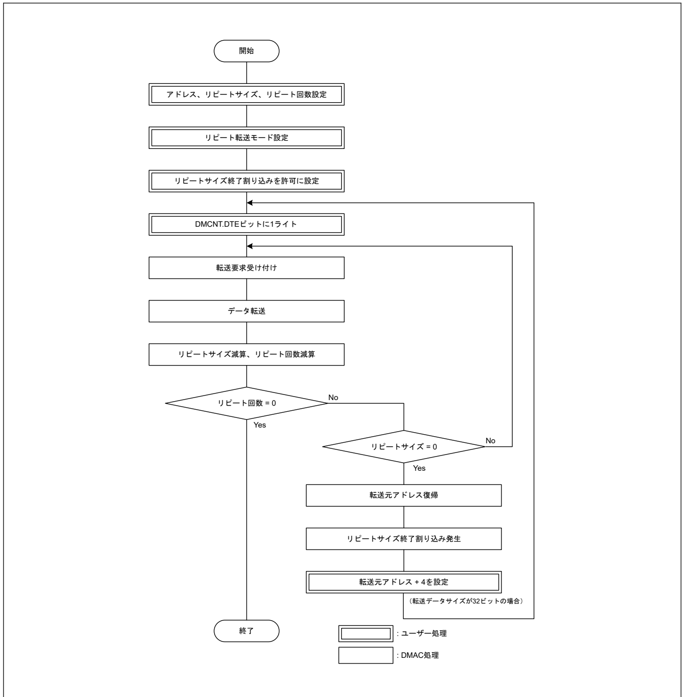
図 16.13 リpeat転送モードにおけるオフセット加算による XY 変換フロー
