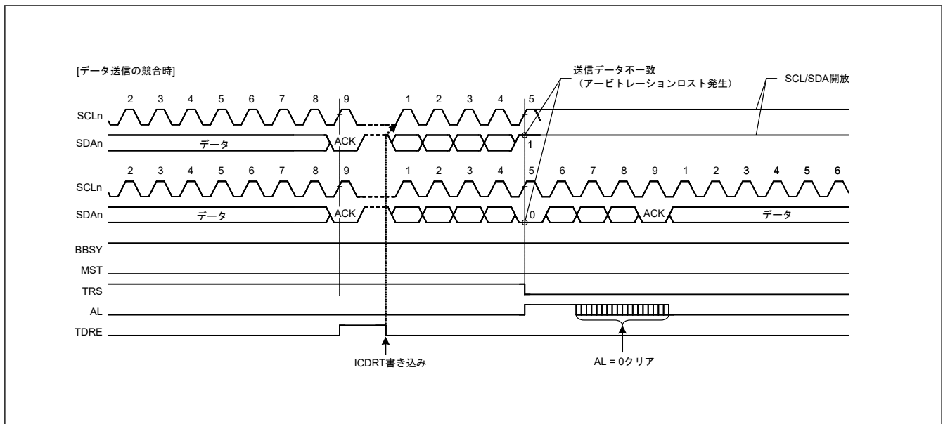
図 30.44 スレーブアービトレーションロスト検出動作例 (SALE = 1 の場合)
