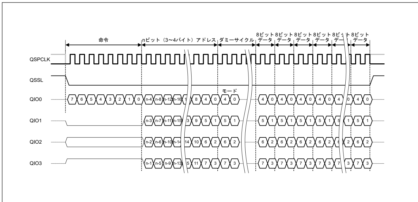
図 33.5 拡張 SPI プロトコル例 (ファストリード Quad I/O)
