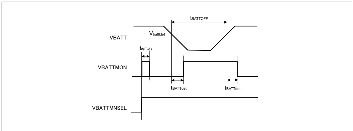
図 47.65 バッテリバックアップ機能特性
