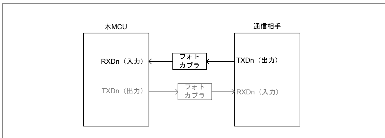
図 29.31 フォトカプラを通過する受信のブロック図イメージ
