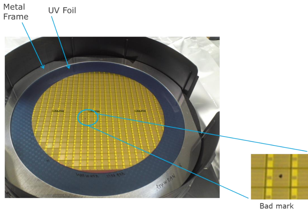
図 5 Sawn wafer 梱包外見 (8 インチウエハ)
