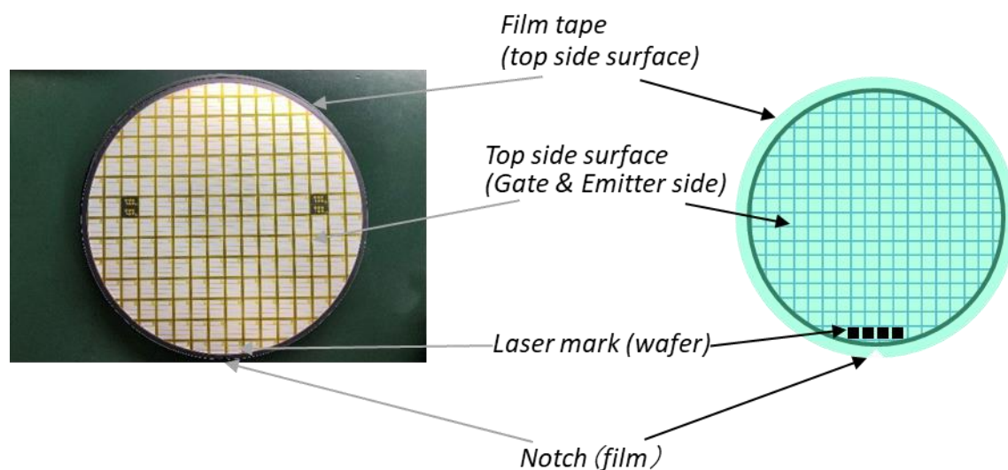
図 9 Unsawn wafer の Laser mark レイアウト
