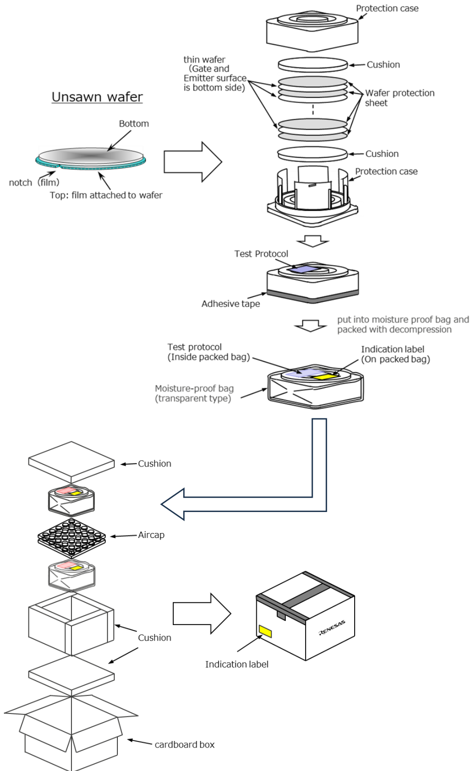
図 7 Unsawn wafer 梱包仕様
