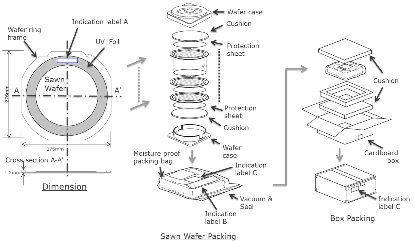
図 1 Sawn Wafer 梱包仕様
