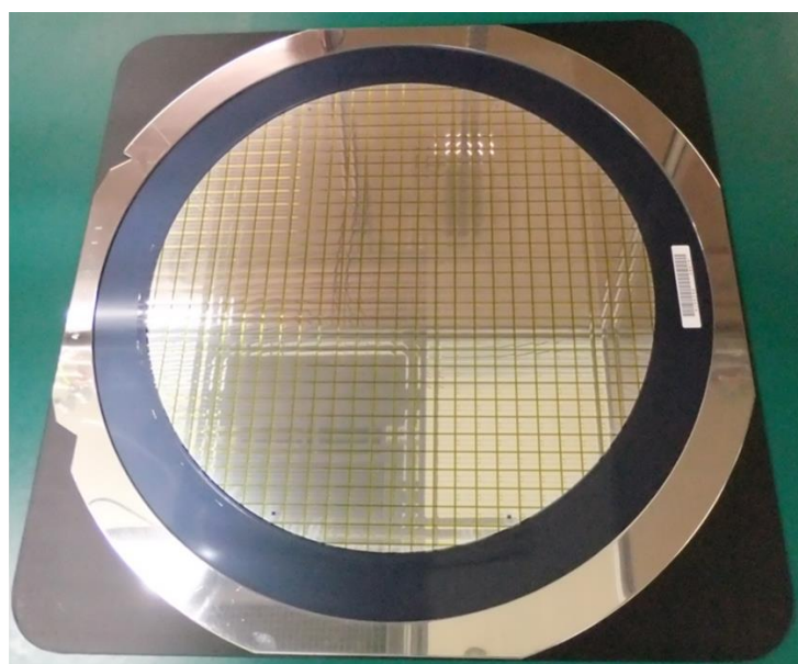
図 6 Sawn wafer 梱包外見 (12 インチウエハ)
