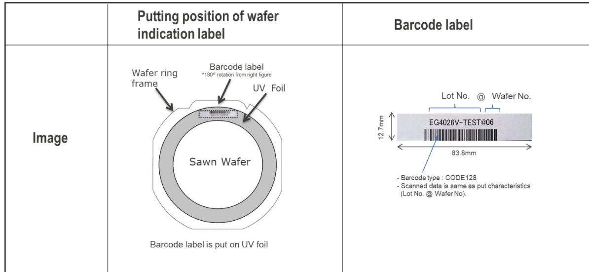
図 3 表示ラベル A
