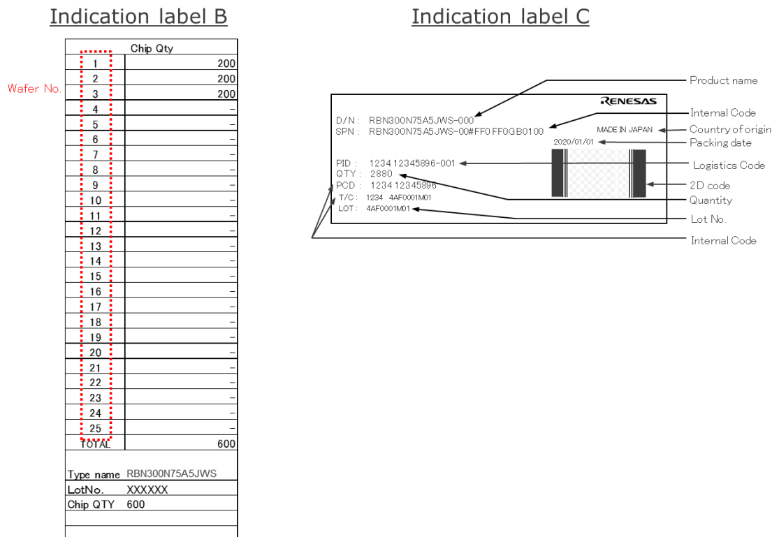
図 4 表示ラベル B,C
