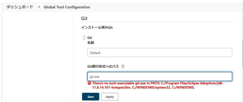
図 14 「There's no such executable git.exe in PATH」 エラー
