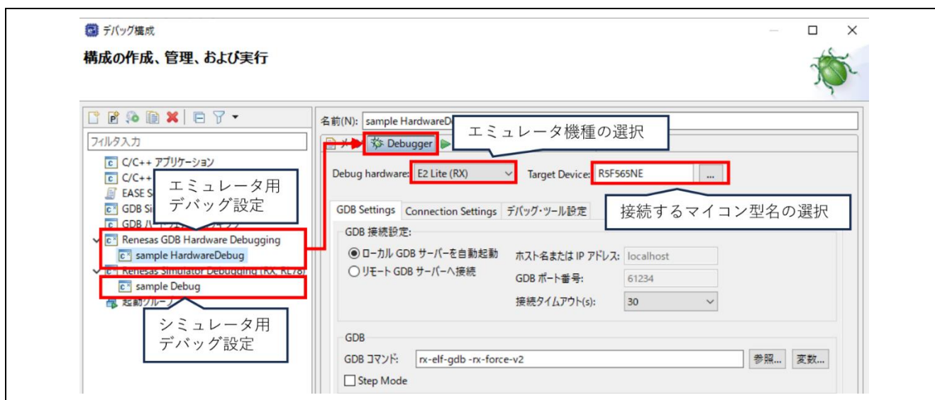
図 4-1 エミュレータ接続の設定箇所
