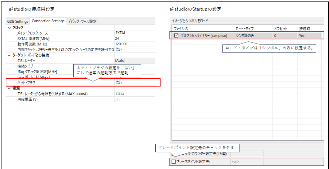
図 5-2 ホットプラグイン接続時の接続用設定
