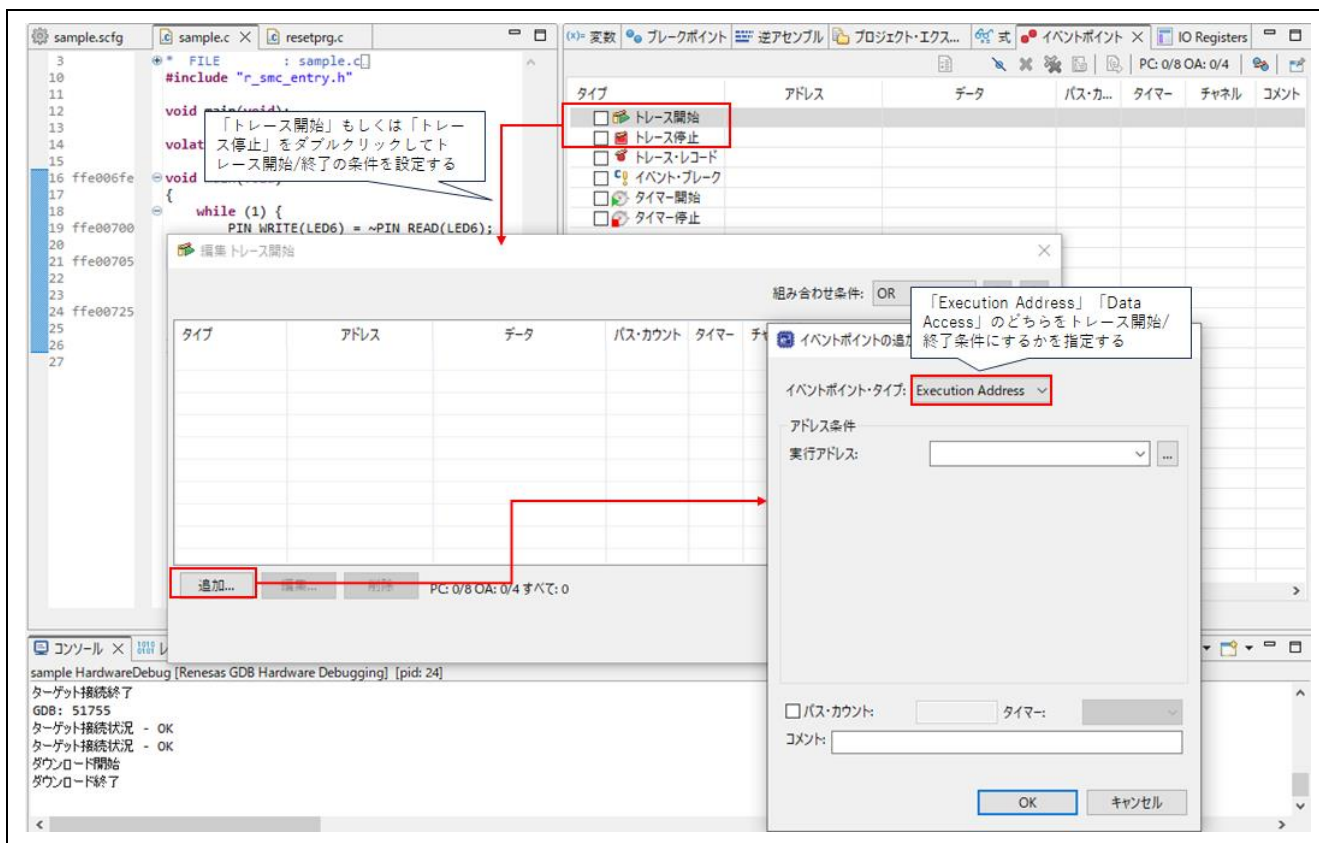
図 6-6 トレースの開始/終了条件の設定
