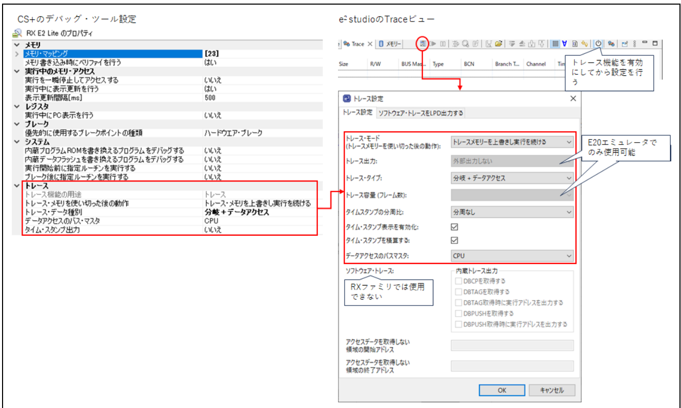
図 6-5 トレースの設定方法
