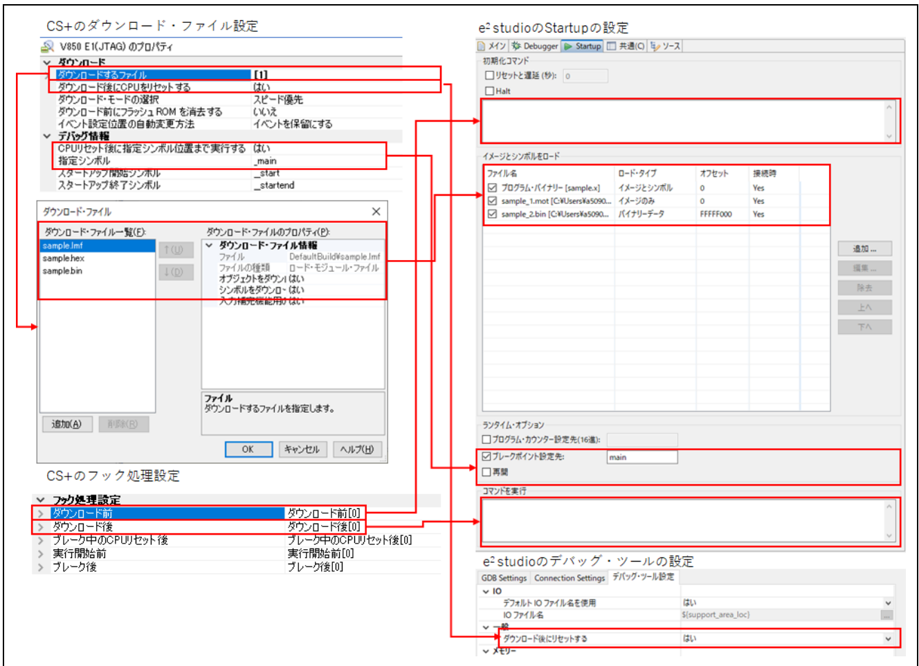
図 5-1 ダウンロードファイルとコマンド処理
