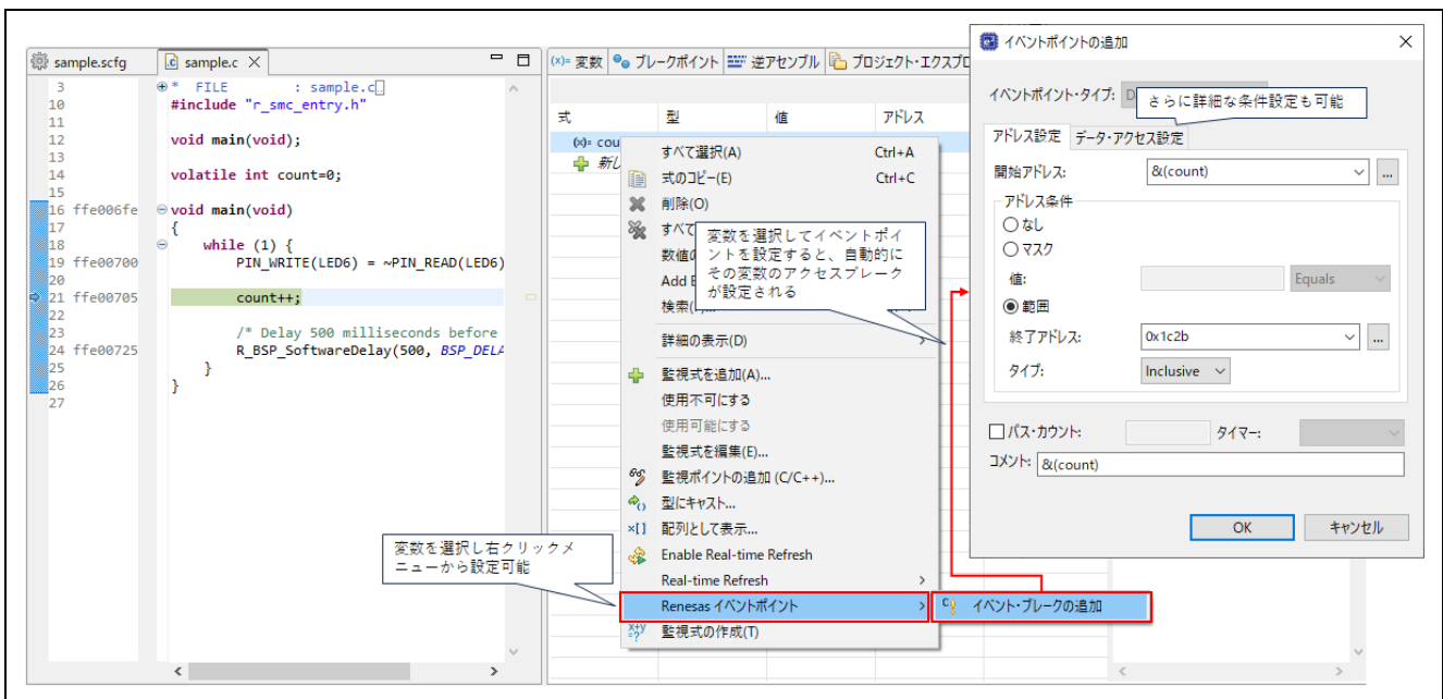
図 6-3 データアクセスブレークの設定方法(1)
