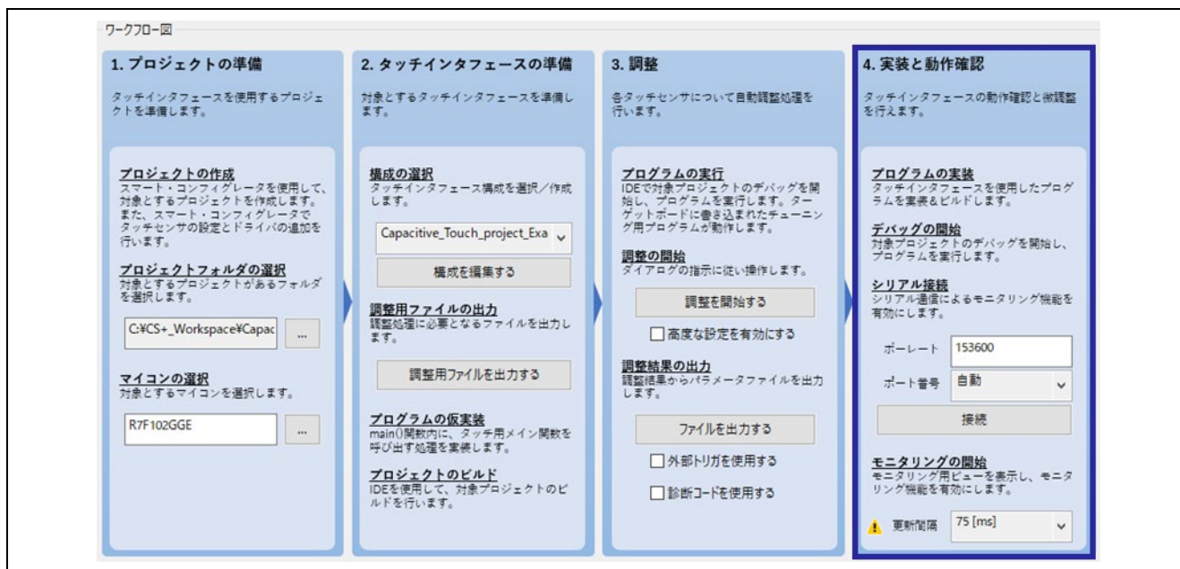
図 8-43 ワークフロー図 (実装と動作確認)
