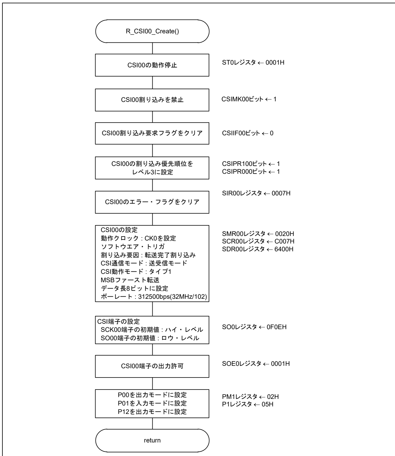
図 5.7 SAU0 チャンネル 0 (CSI00) の動作設定
