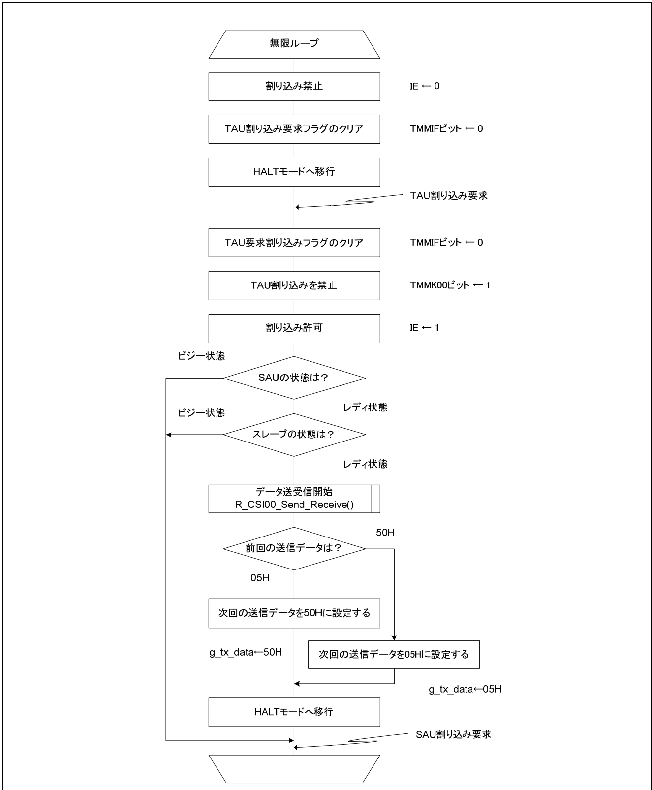
図 5.12 メイン処理内の無限ループ
