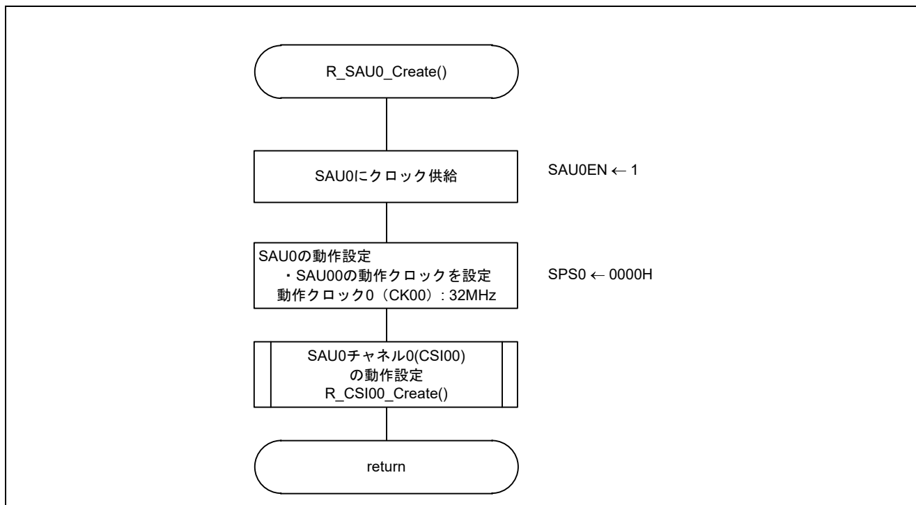
図 5.6 SAU0 の設定
