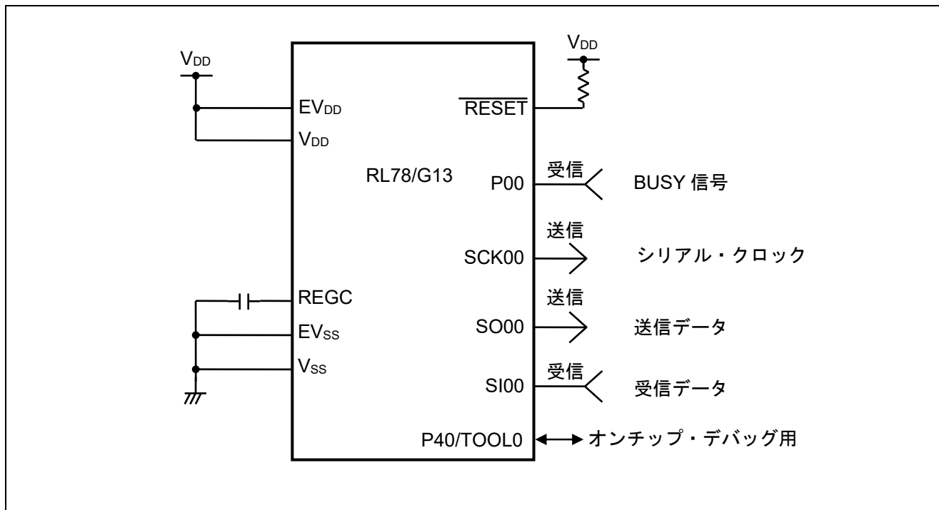
図 4.2 ハードウェア構成
