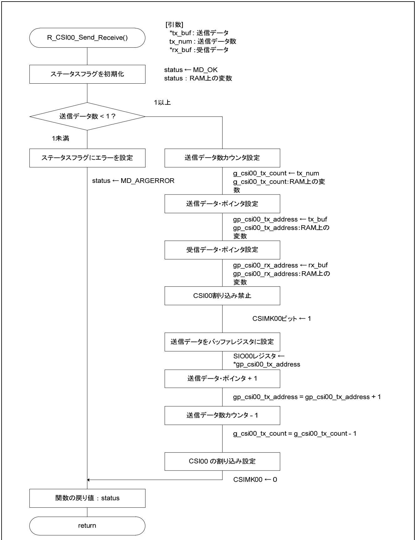
図 5.13 CSI00 データ送受信開始処理
