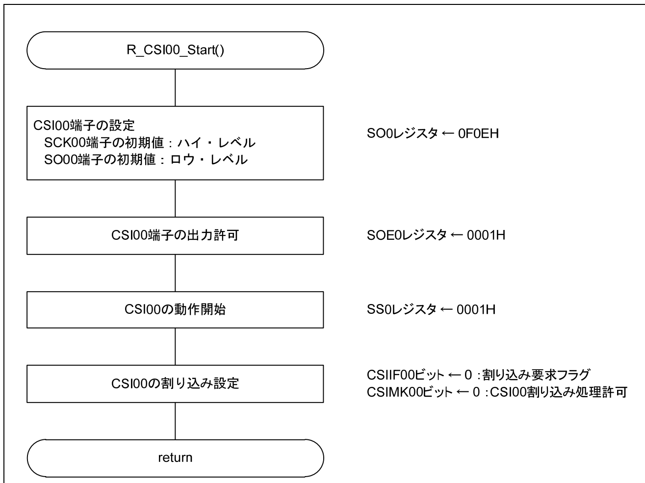
図 5.11 SAU0 チャンネル 0 (CSI00) の動作開始処理
