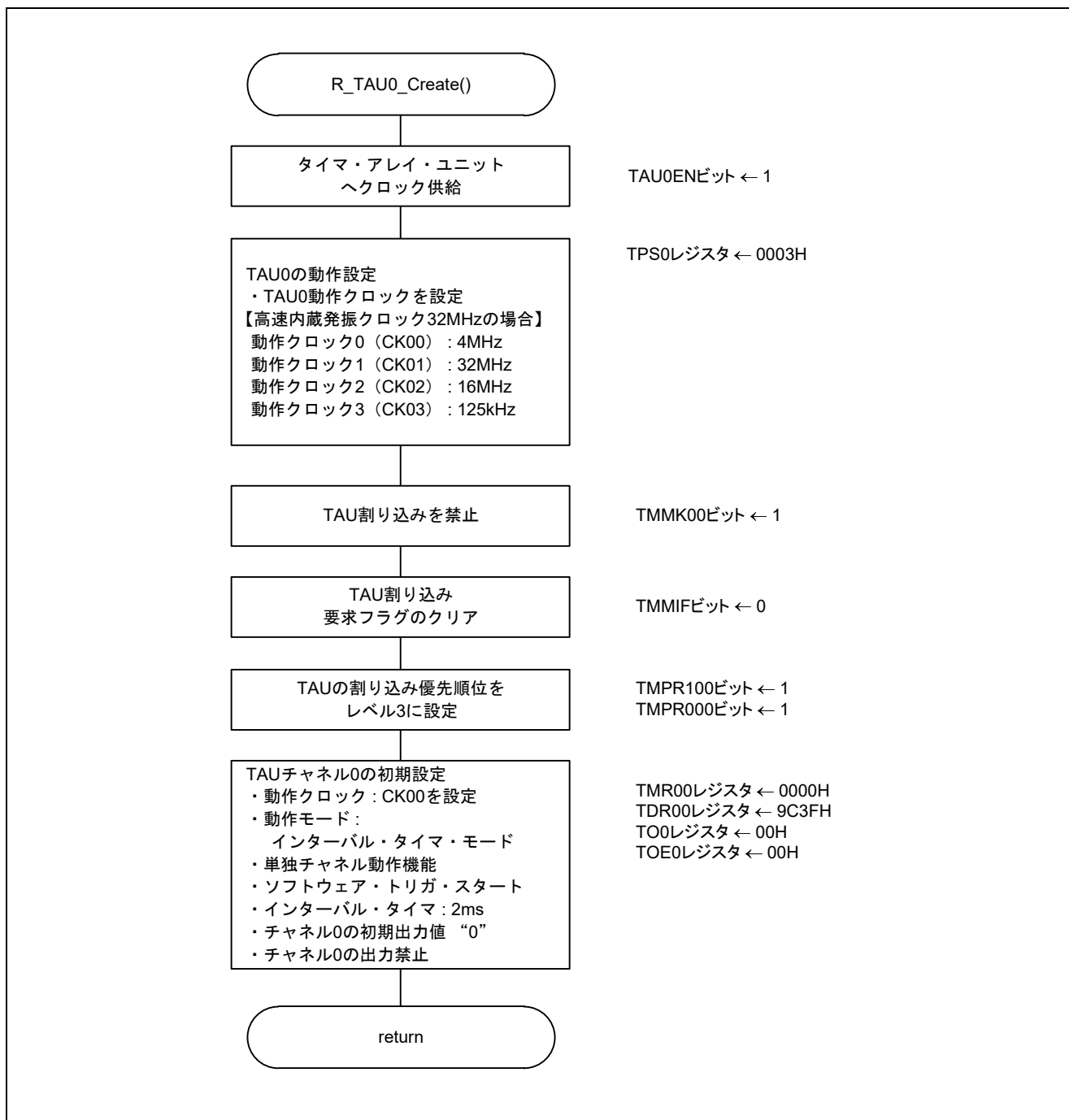
図 5.8 TAU0 の設定
