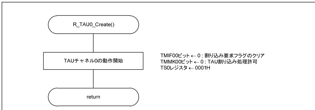
図 5.10 TAU0 チャンネル 0 の動作開始処理
