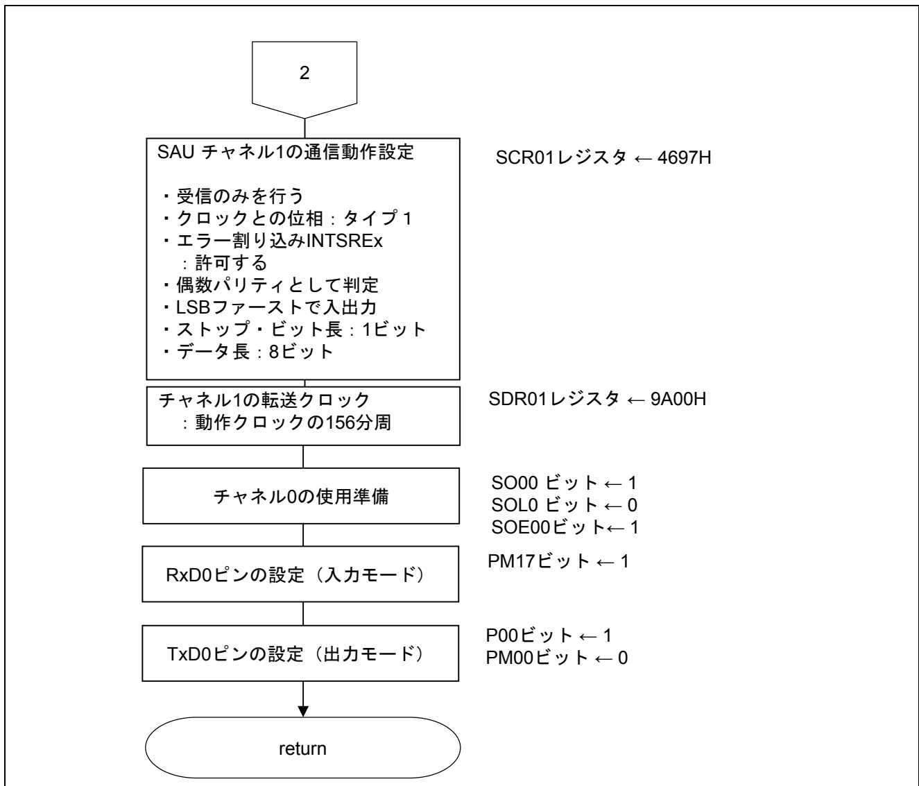
図 5.9 UART0 の設定 (3/3)
