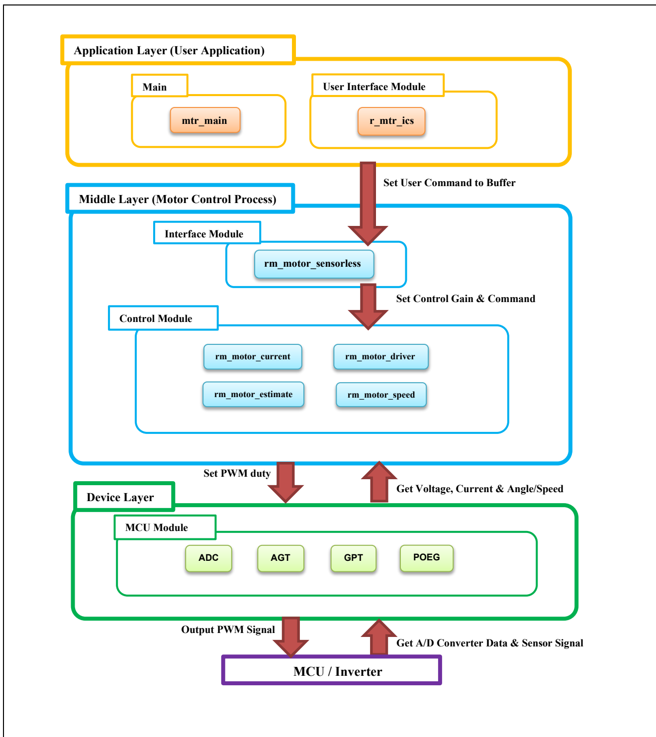
図 2-21 モジュール構成
