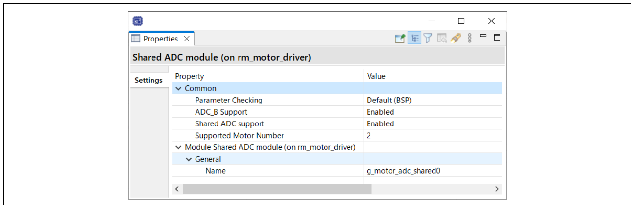
図 2-6 ADC シェアードモジュールの FSP コンフィグレーション
