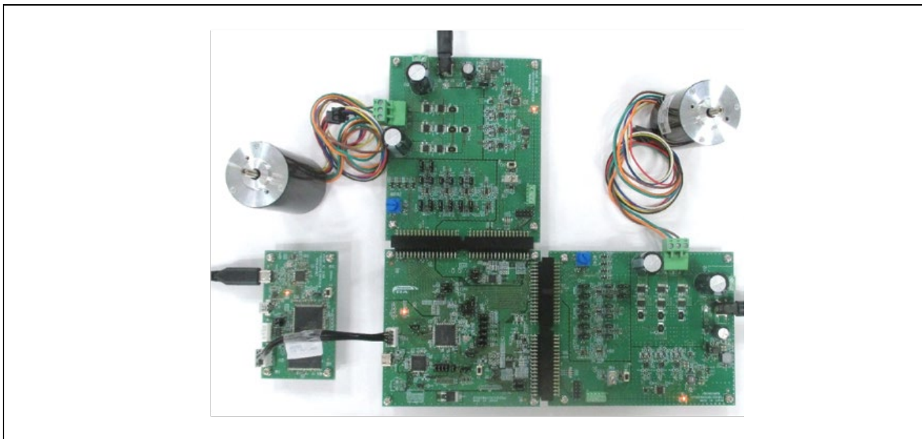
図 2-4 CPU ボードとインバータボードの接続
