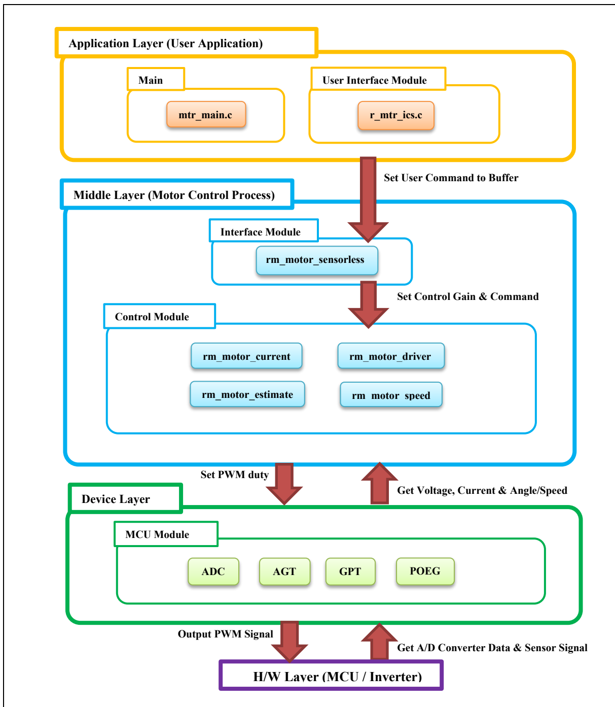
図 2-27 モジュール構成
