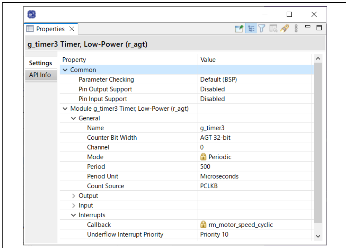
図 2-6 AGT ドライバの FSP コンフィグレーション
