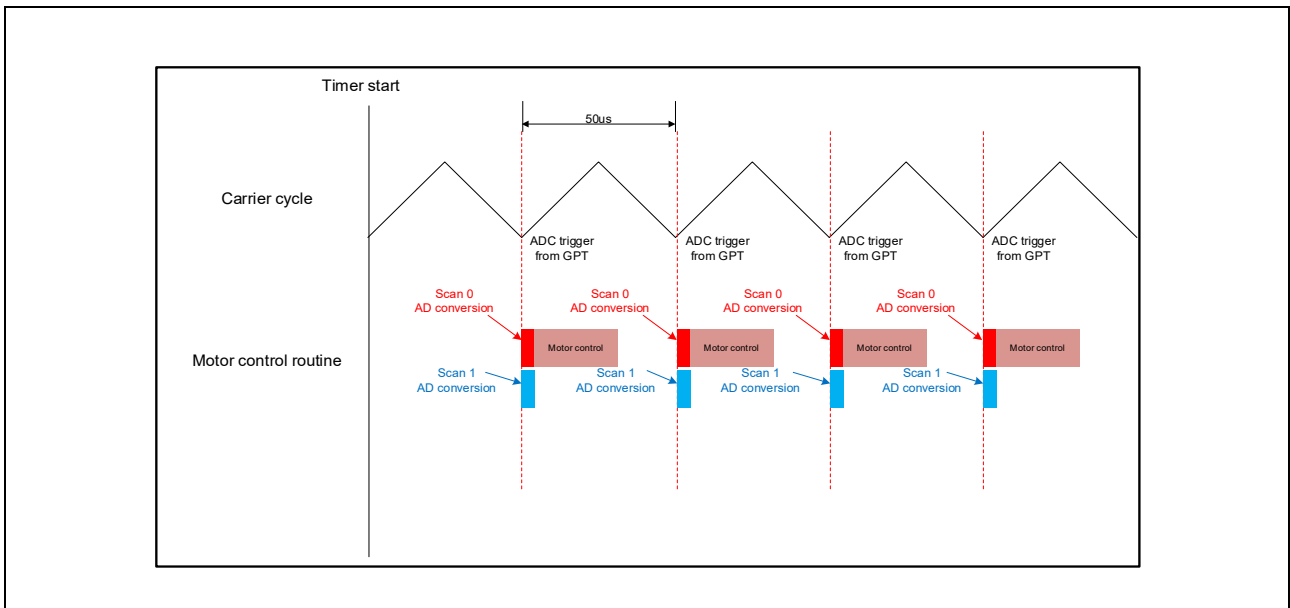
図 3-3 AD トリガタイミング
