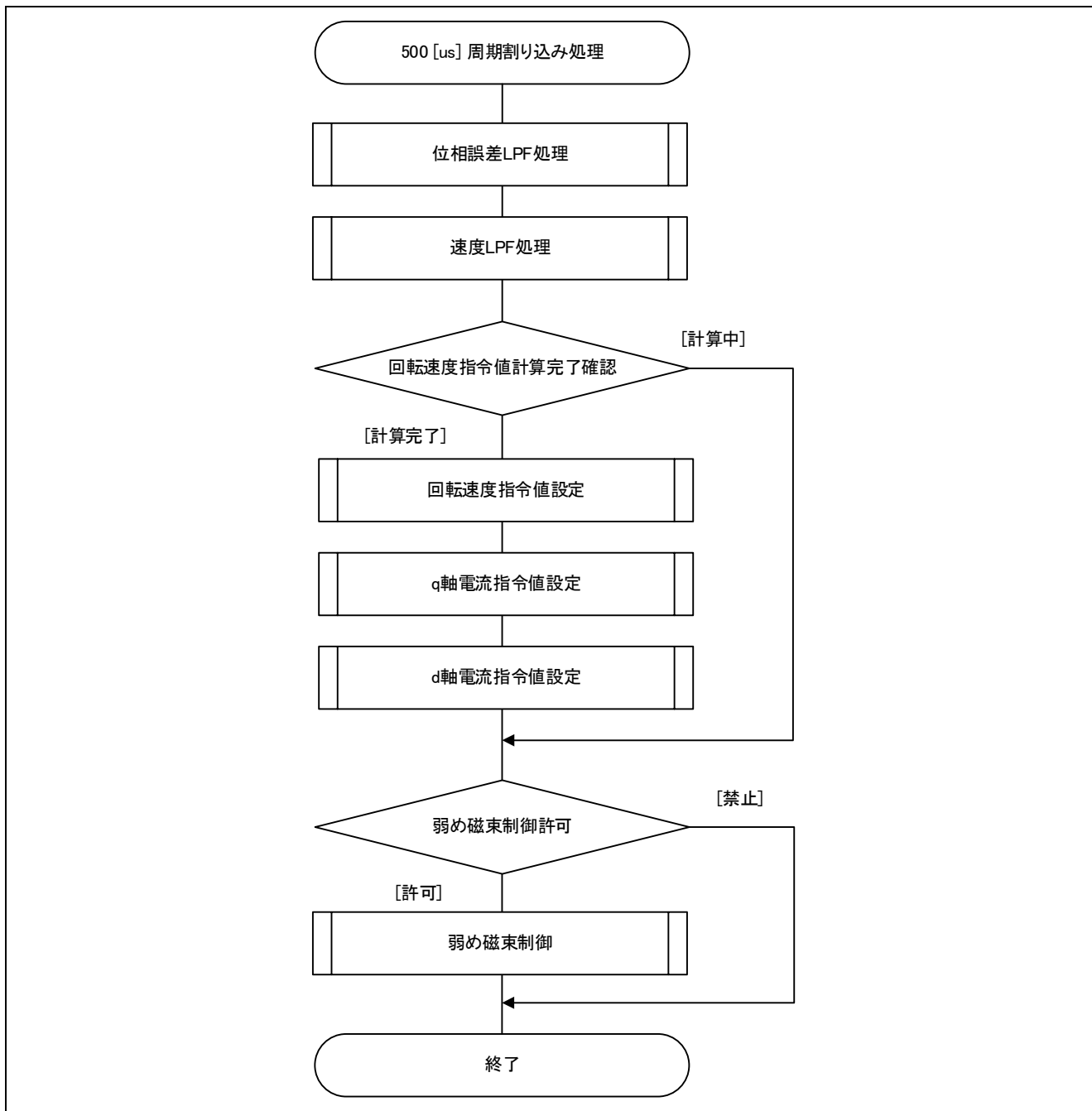
図 3-9 速度制御周期割り込み処理フローチャート
