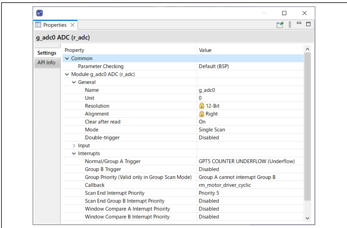
図 2-22 ADC ドライバの FSP コンフィグレーション [1/2]
