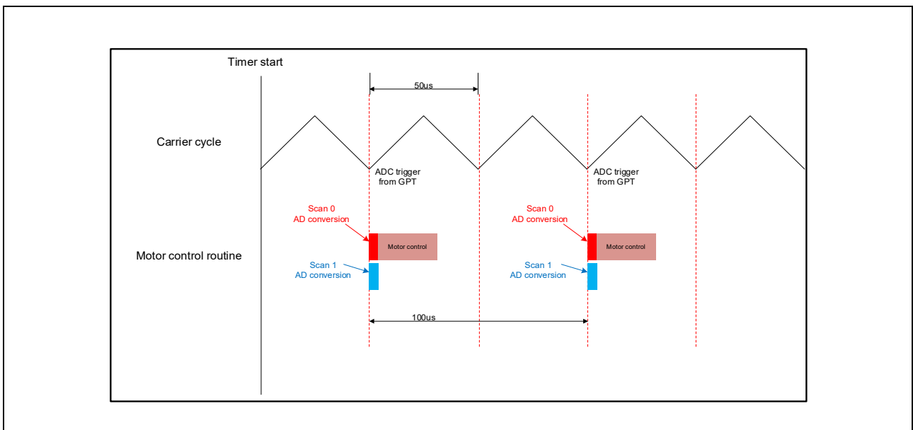
図 3-4 AD トリガタイミング(1 回間引き)
