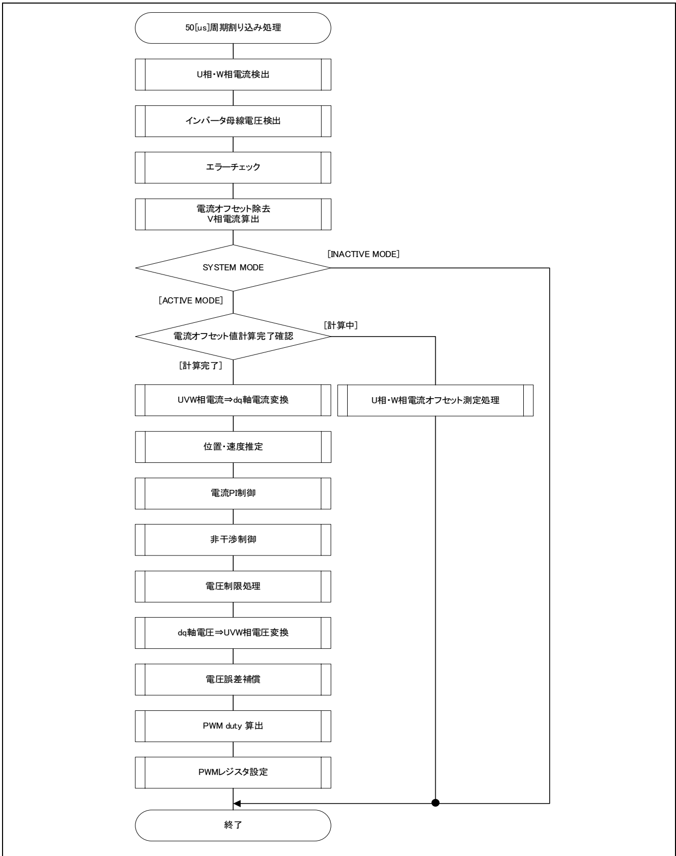
図 3-8 電流制御周期割り込み処理フローチャート
