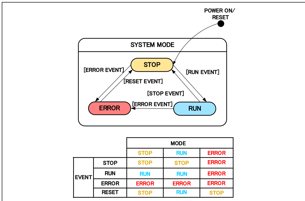
図 3-1 センサレスベクトル制御ソフトウェアの状態遷移図
