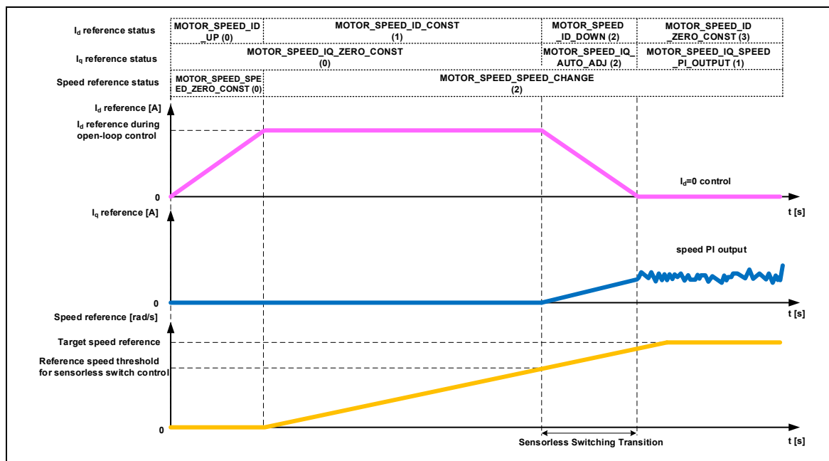
図 3-2 センサレスベクトル制御ソフトウェアの始動制御内容
