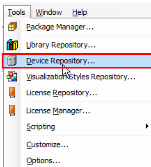
図 2.4 Device Repository
