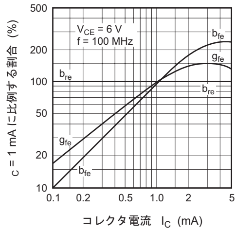
転送アドミタンス対コレクタ電流特性
