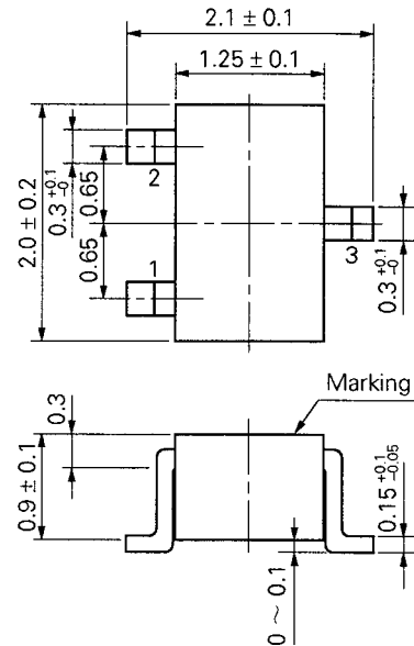
外形図 (単位: mm)
