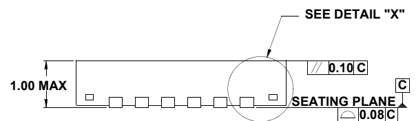
側面図
