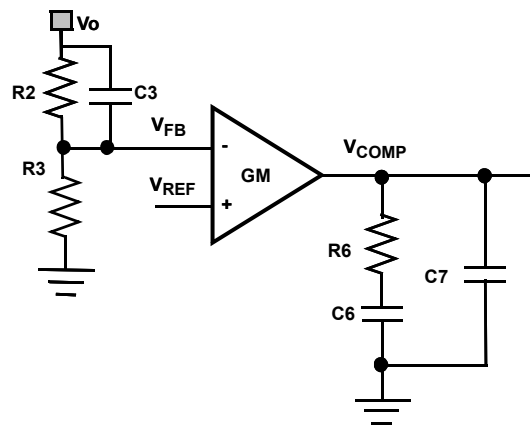
図 48. タイプ II 補償回路
