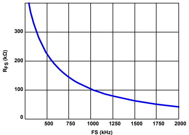
図 46. R_{FS} vs スwitching周波数
