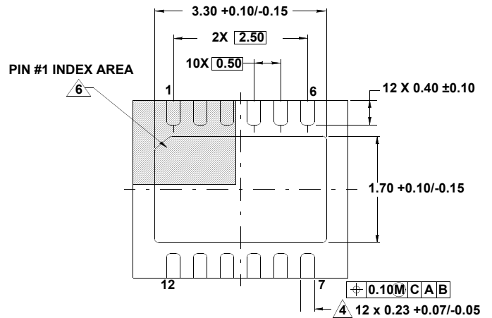
底面図
