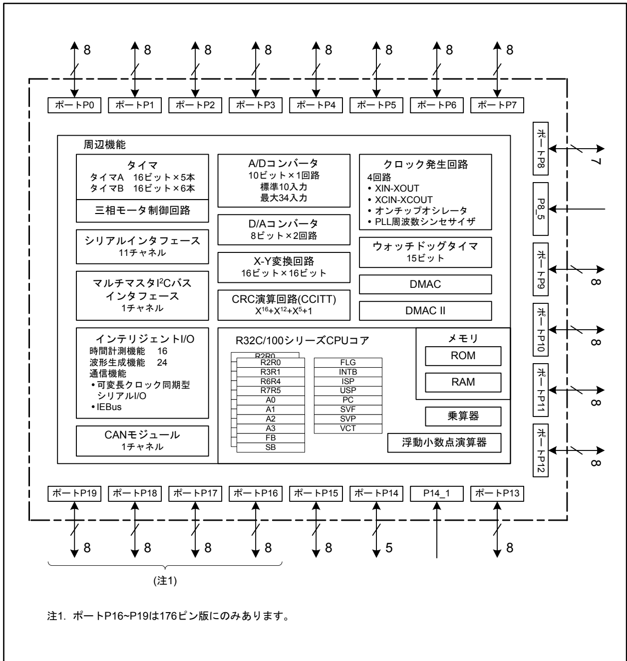
図 1.2 R32C/117A グループのブロック図
