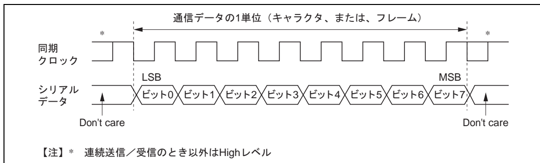
図 14.14 クロック同期式通信のデータフォーマット
