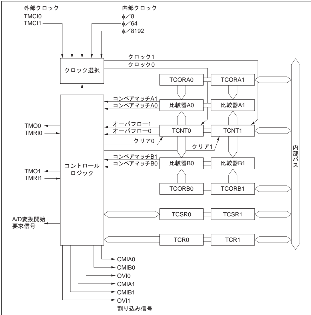
図 12.1 8ビットタイマのブロック図
