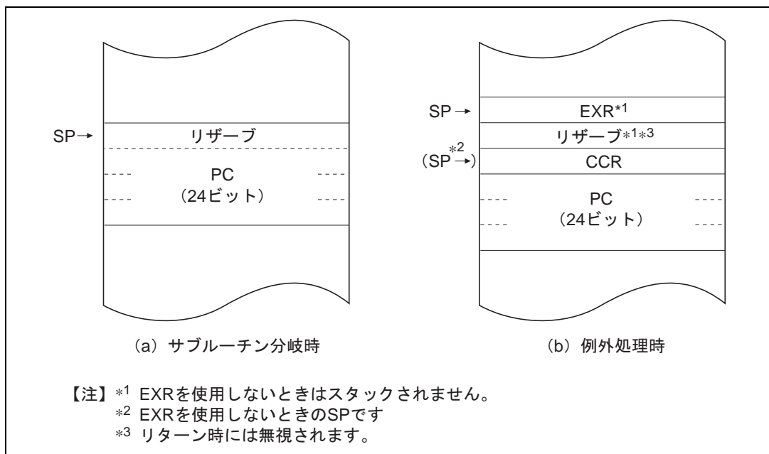
図 2.2 アドバンストモードのスタック構造
