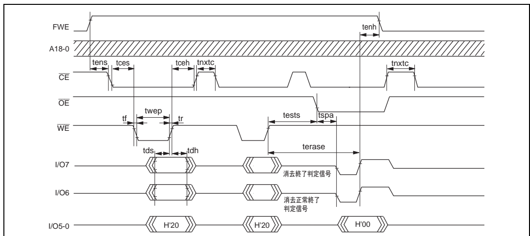
図 19.53 自動消去モードのタイミング波形
