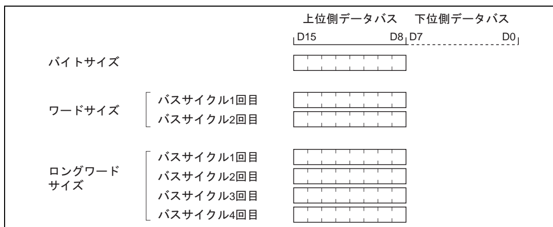
図 6.4 アクセスサイズとデータアライメント制御 (8 ビットアクセス空間)
