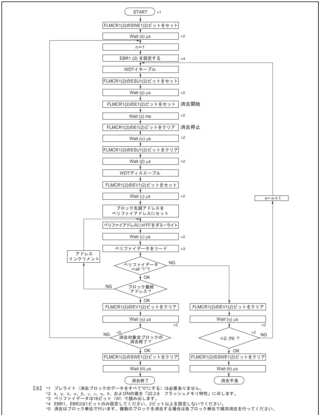
図 19.72 イレース/イレースペリファイフロー
