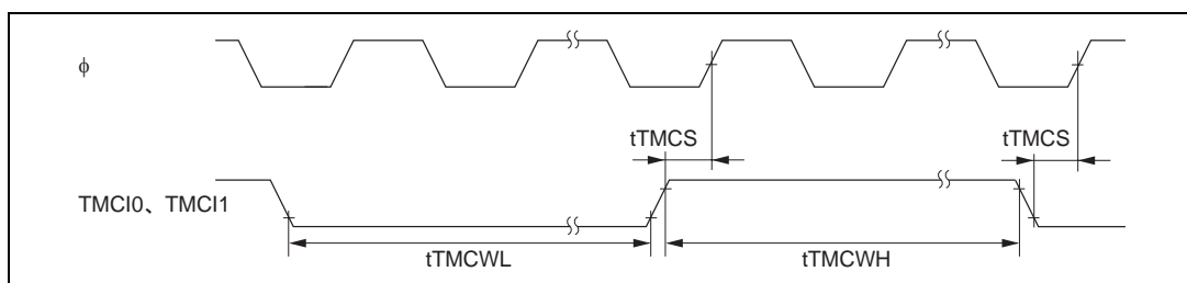
図 22.25 8ビットタイマクロック入力タイミング
