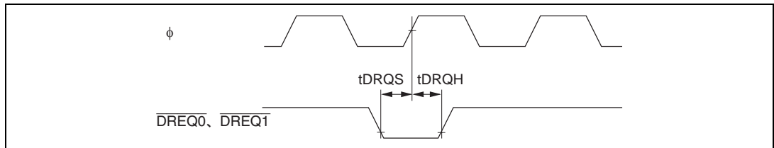
図 22.19 DMAC \overline{\text{DREQ}} 入力タイミング
