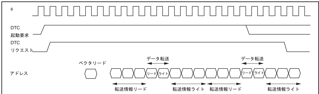
図 8.12 DTC の動作タイミング (チェーン転送の例)
