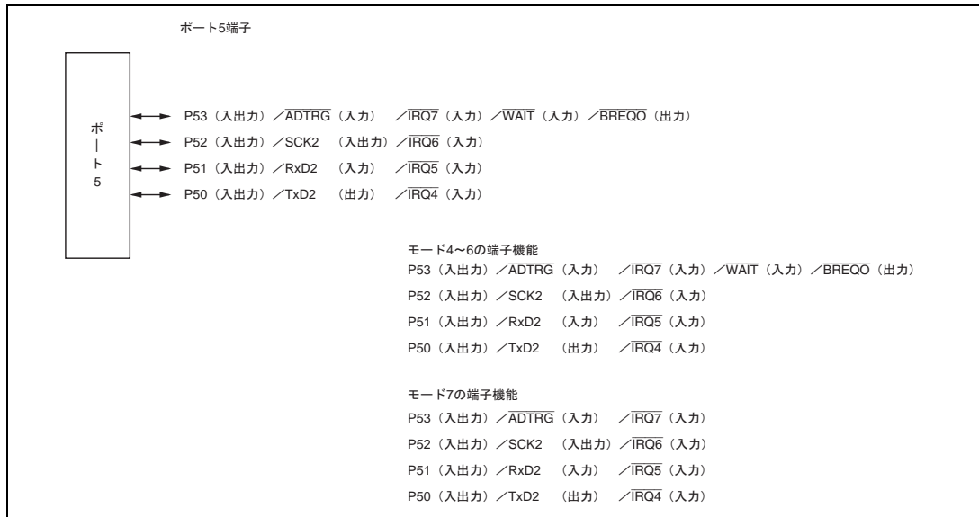
図 9.5 ポート 5 の端子機能
