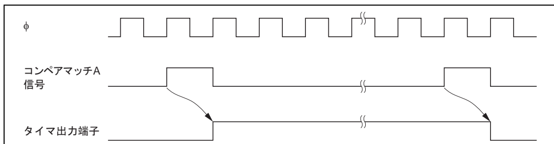
図 12.5 タイマ出力タイミング
