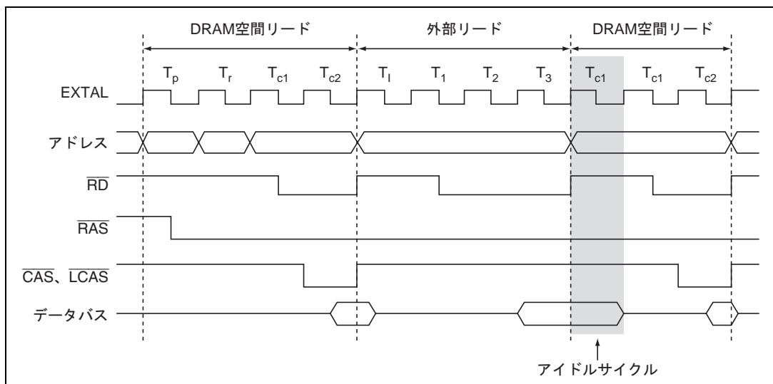
図 6.35 (a) RAS ダウンモード時のアイドルサイクル動作例 (ICIS1 = 1)
