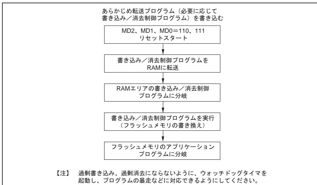
図 19.13 ユーザプログラムモードの実行手順例
