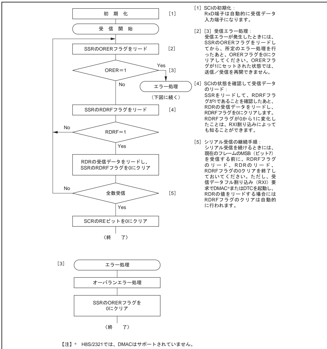
図 14.18 シリアルデータ受信フローチャートの例
