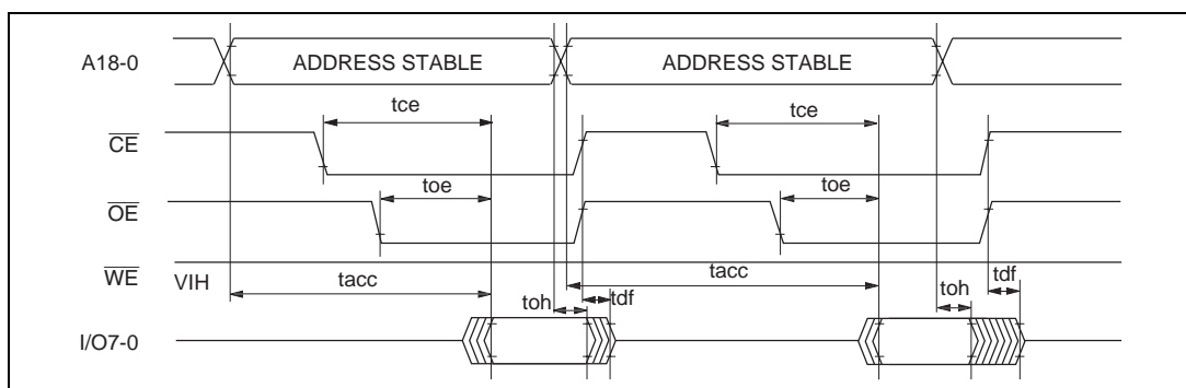
図 19.24 \overline{\text{CE}} 、 \overline{\text{OE}} クロック方式リード時のタイミング波形
