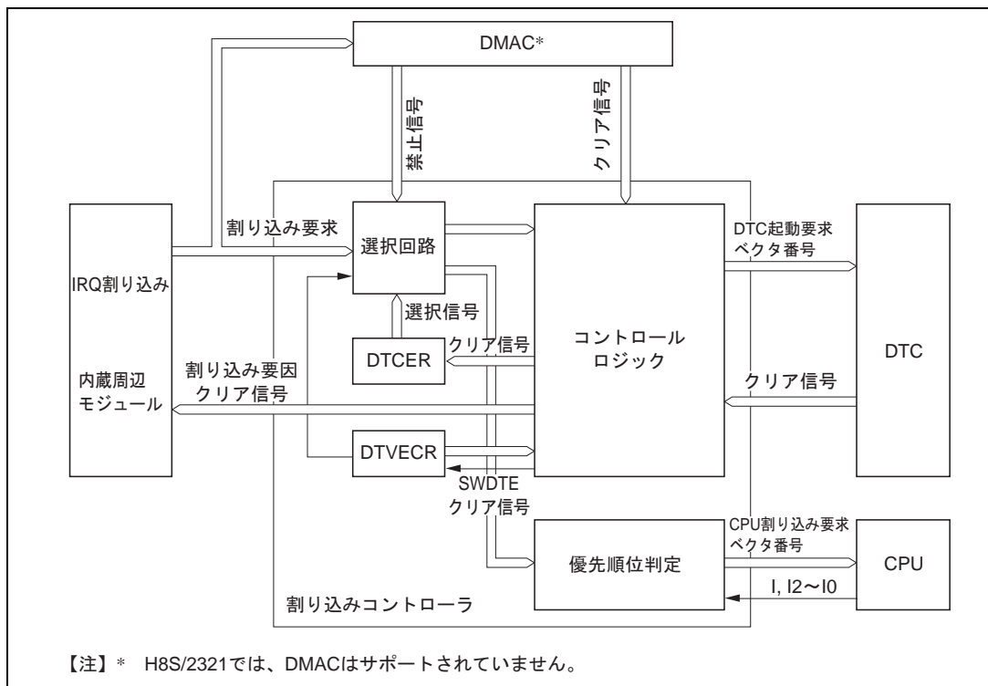
図 5.9 DTC、DMAC と割り込み制御
