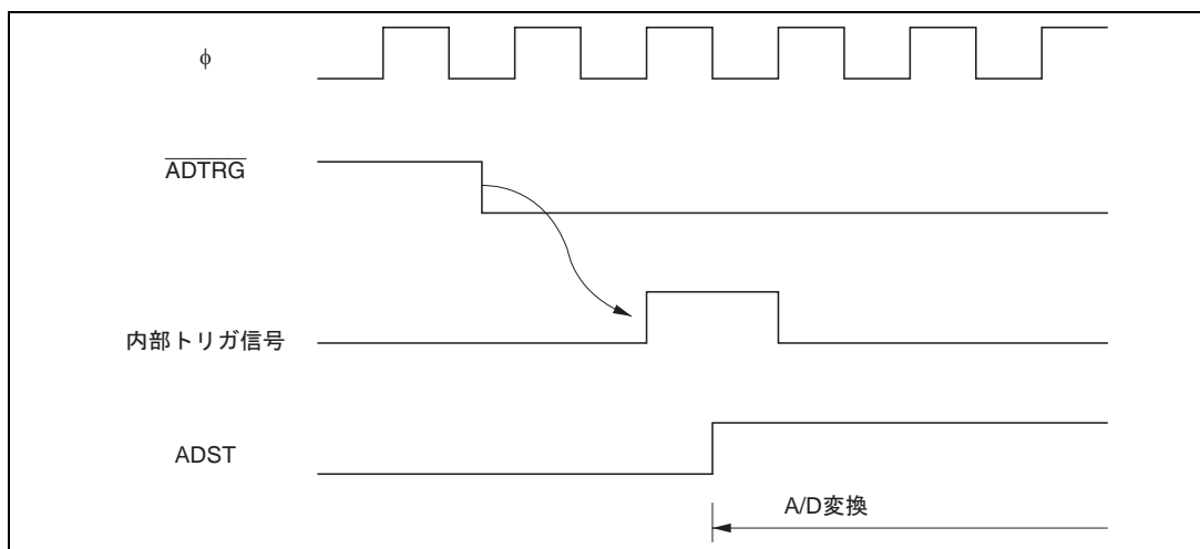
図 16.6 外部トリガ入力タイミング
