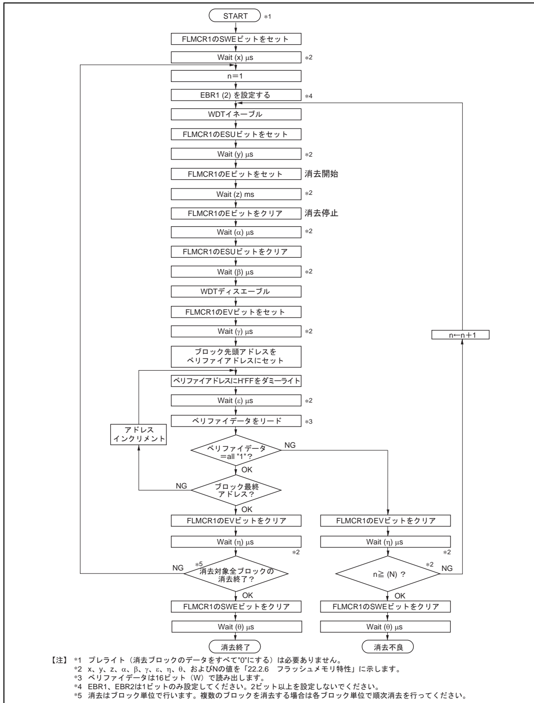
図 19.15 イレース/イレースペリファイフロー
