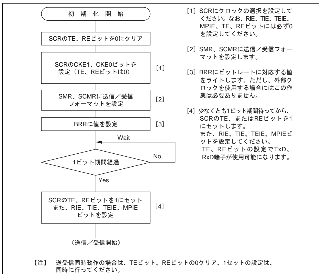
図 14.15 SCI の初期化フローチャートの例
