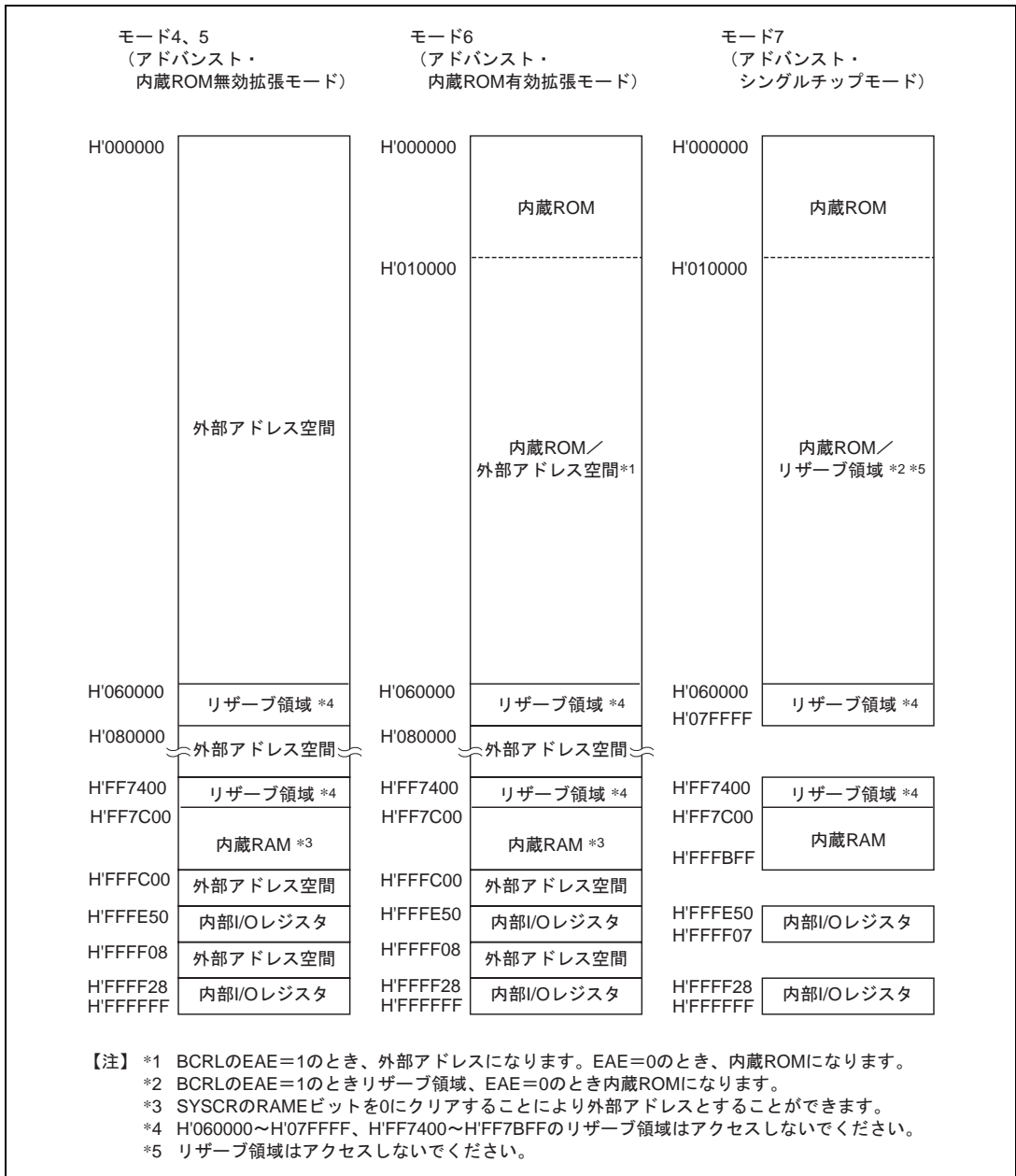
図 3.1 H8S/2329B の各動作モードのアドレスマップ (2)
