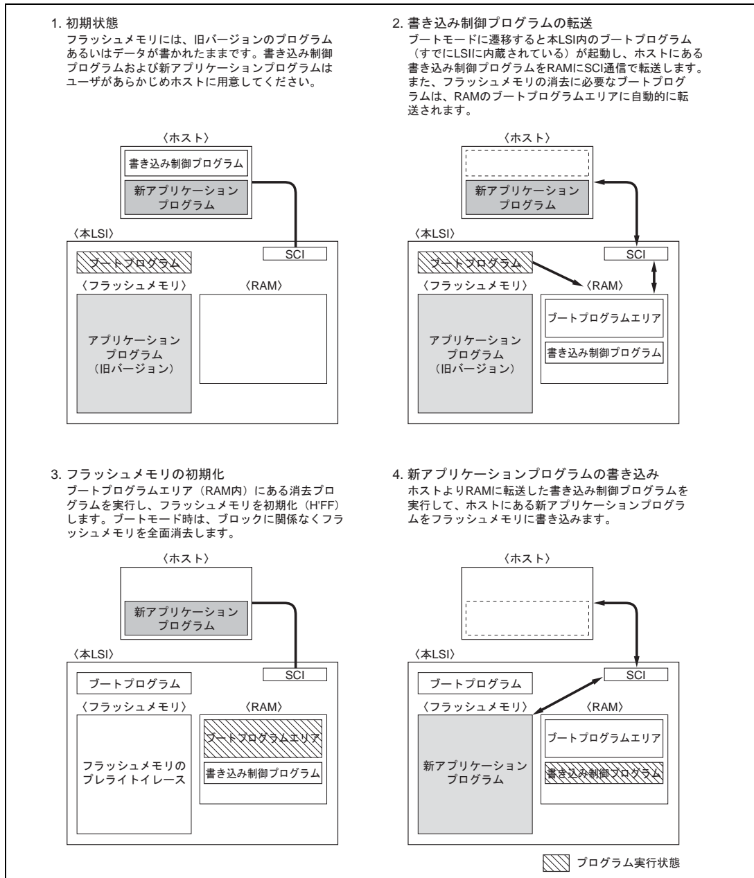
図 19.4 オンボードプログラミング・ブートモード
