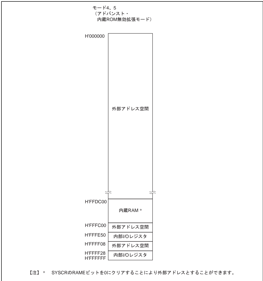
図 3.7 H8S/2322R の各動作モードのアドレスマップ
