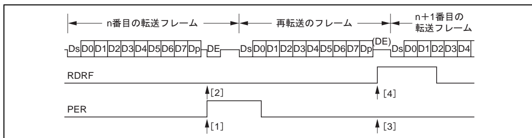
図 15.11 SCI 受信モードの場合の再転送動作
