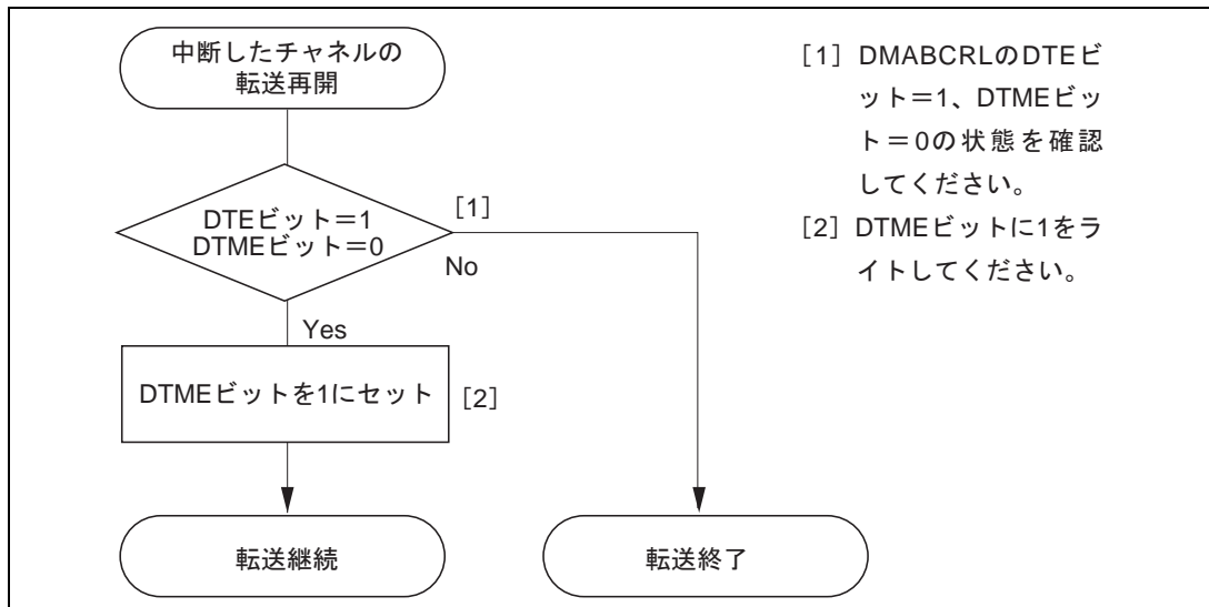
図 7.36 NMI 割り込みにより中断したチャンネルの転送継続手順例
