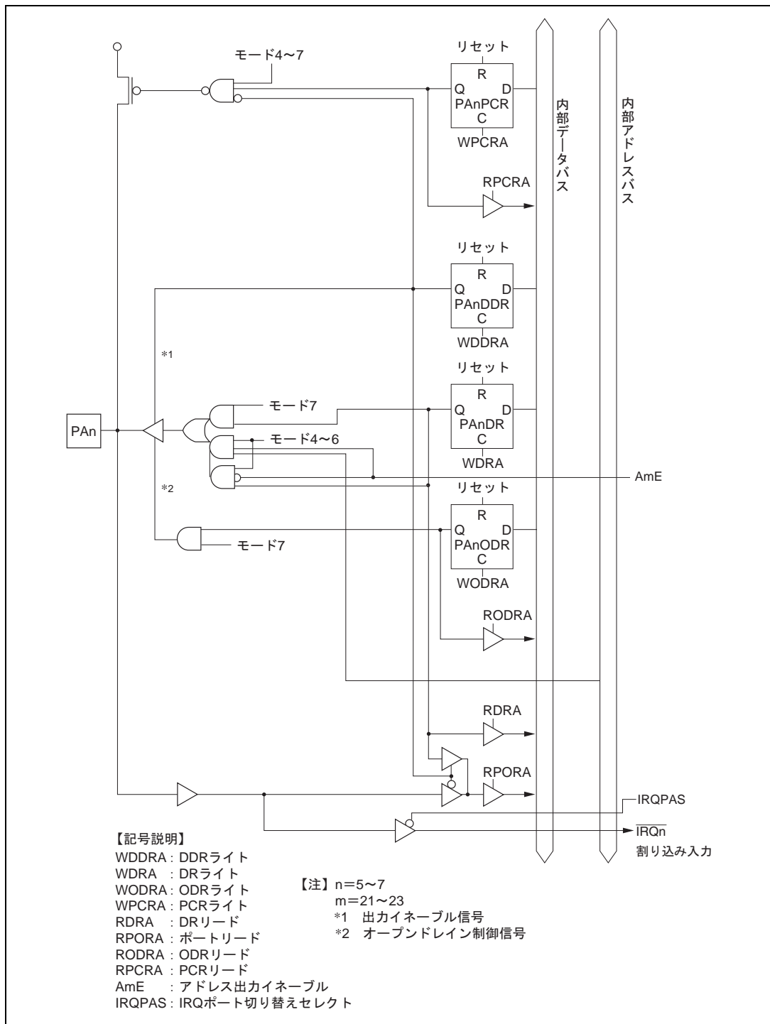
図 C.7 (c) ポート A ブロック図 (PA5 ~ PA7 端子)
