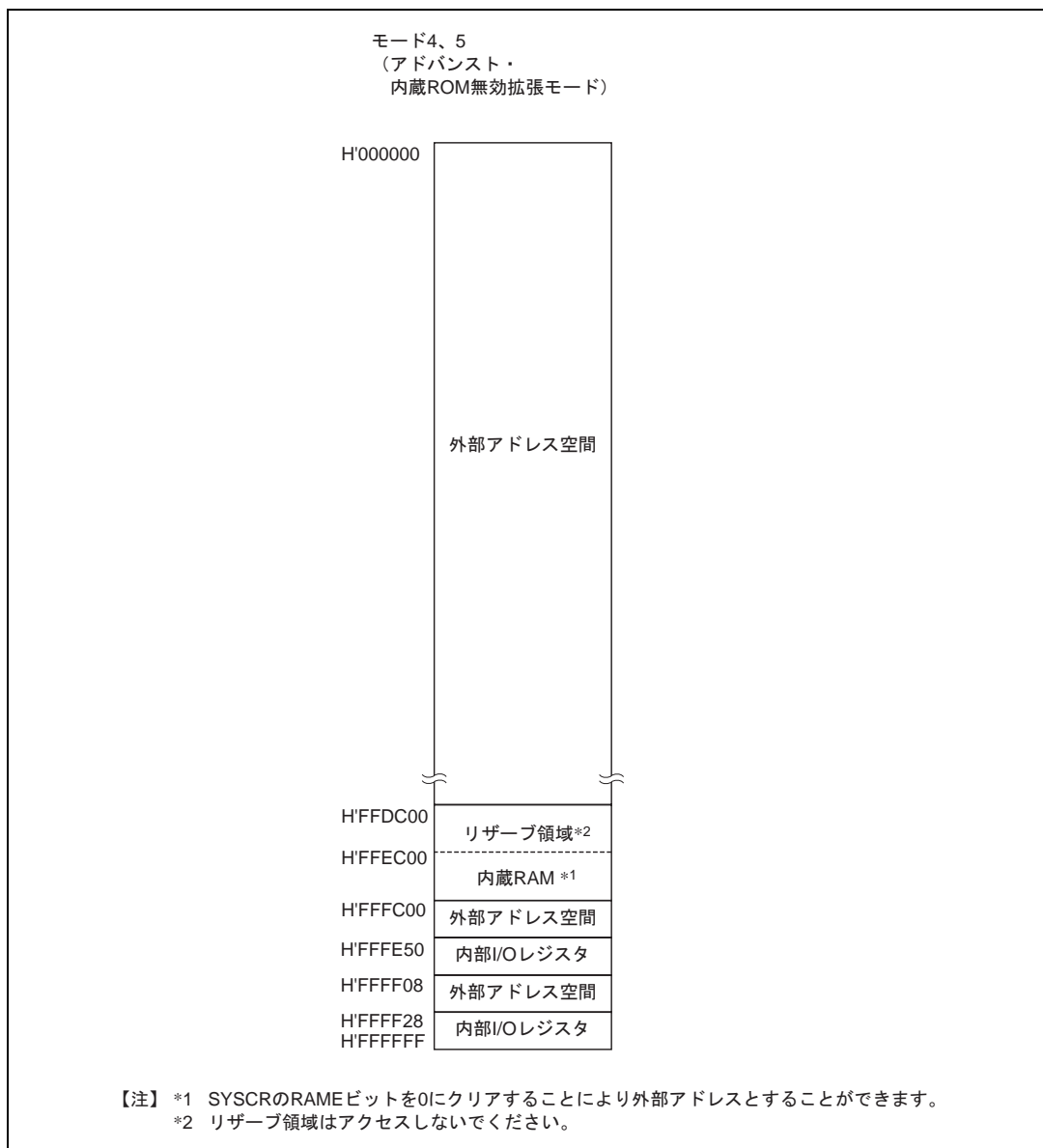
図 3.8 H8S/2320、H8S/2321 の各動作モードのアドレスマップ
