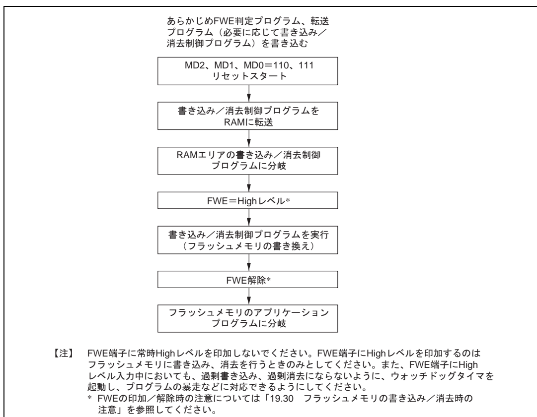
図 19.70 ユーザプログラムモードの実行手順例
