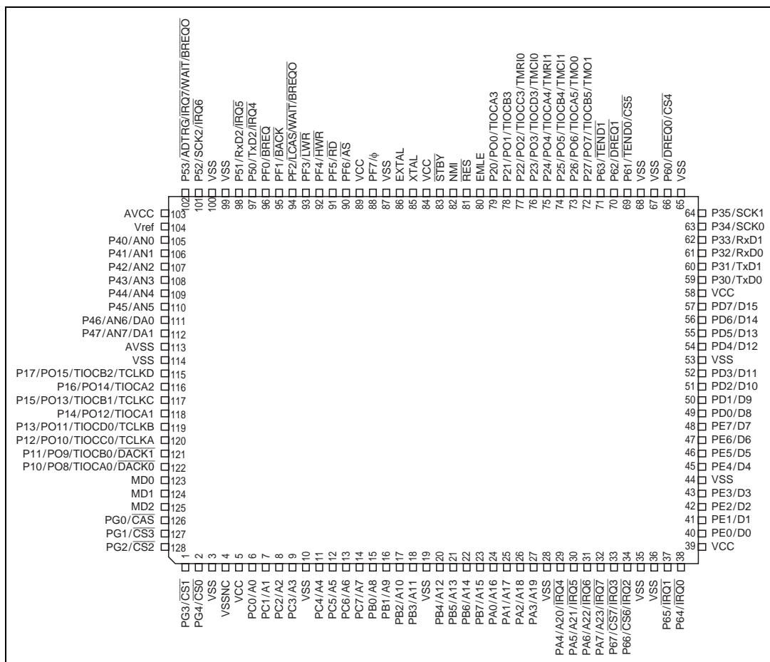
図 1.8 HD64F2329B ピン配置図 (FP-128B : 上面図)
