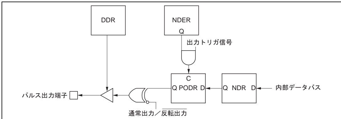
図 11.2 PPG 出力動作
