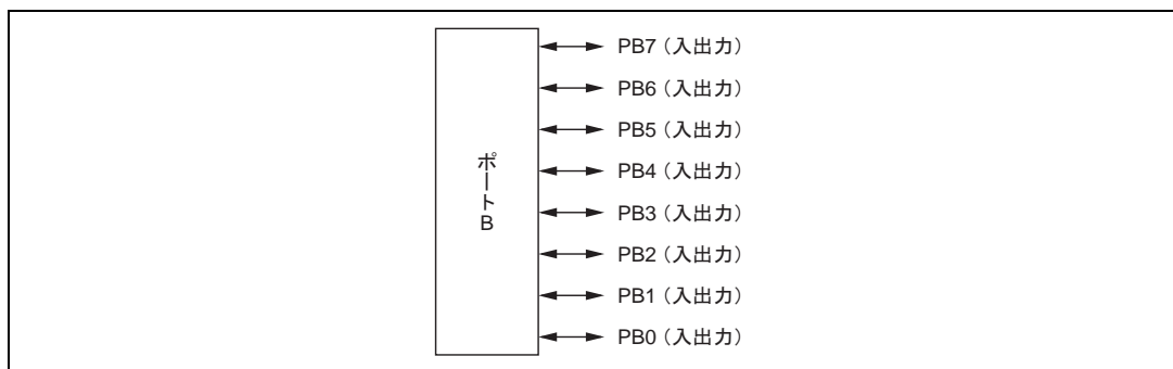
図 9.11 ポート B の端子機能 (モード 7)
