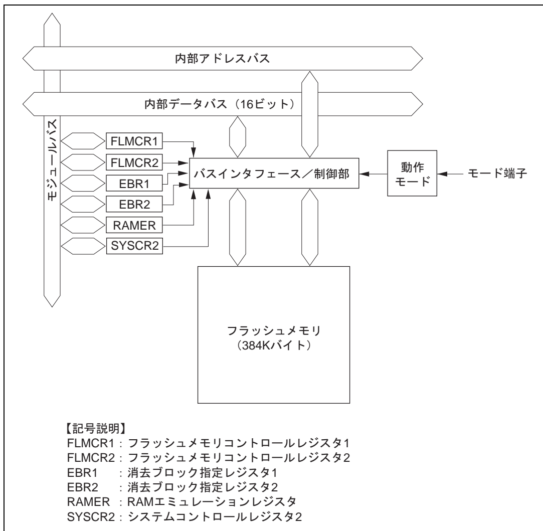
図 19.2 フラッシュメモリのブロック図
