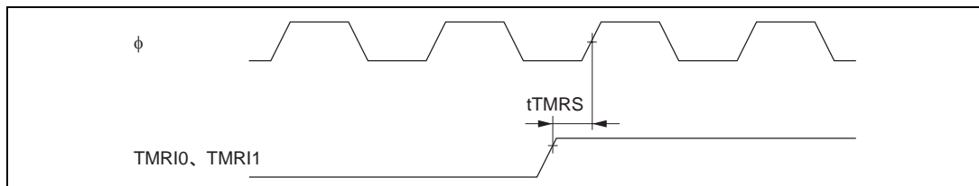
図 22.26 8ビットタイマリセット入力タイミング
