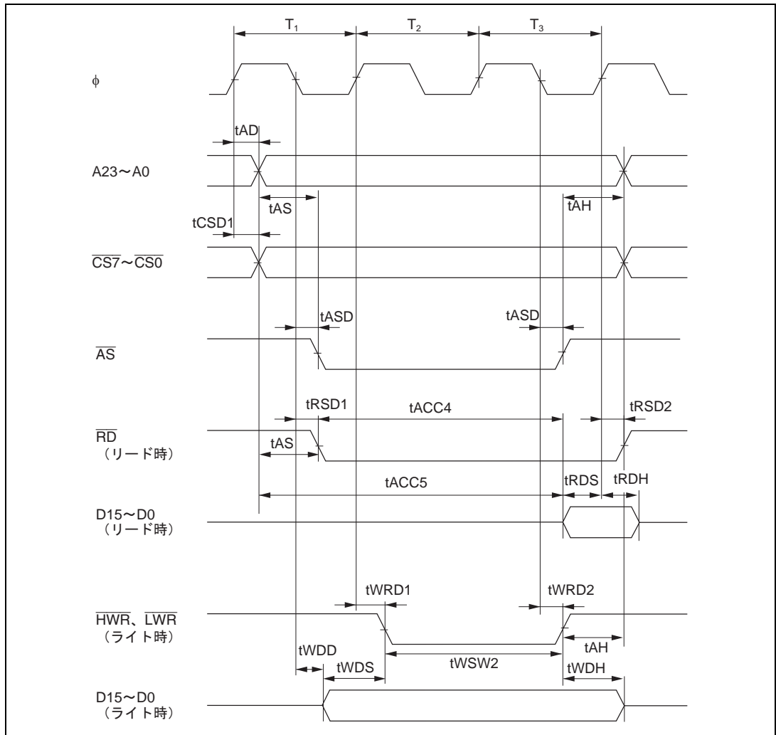
図 22.7 基本バスタイミング / 3 ステートアクセス
