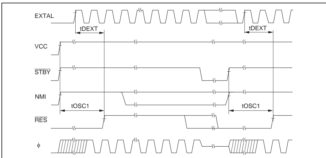
図 22.3 発振安定時間タイミング
