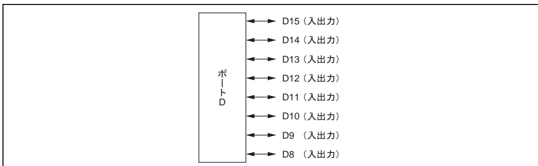
図 9.17 ポート D の端子機能 (モード 4~6)
