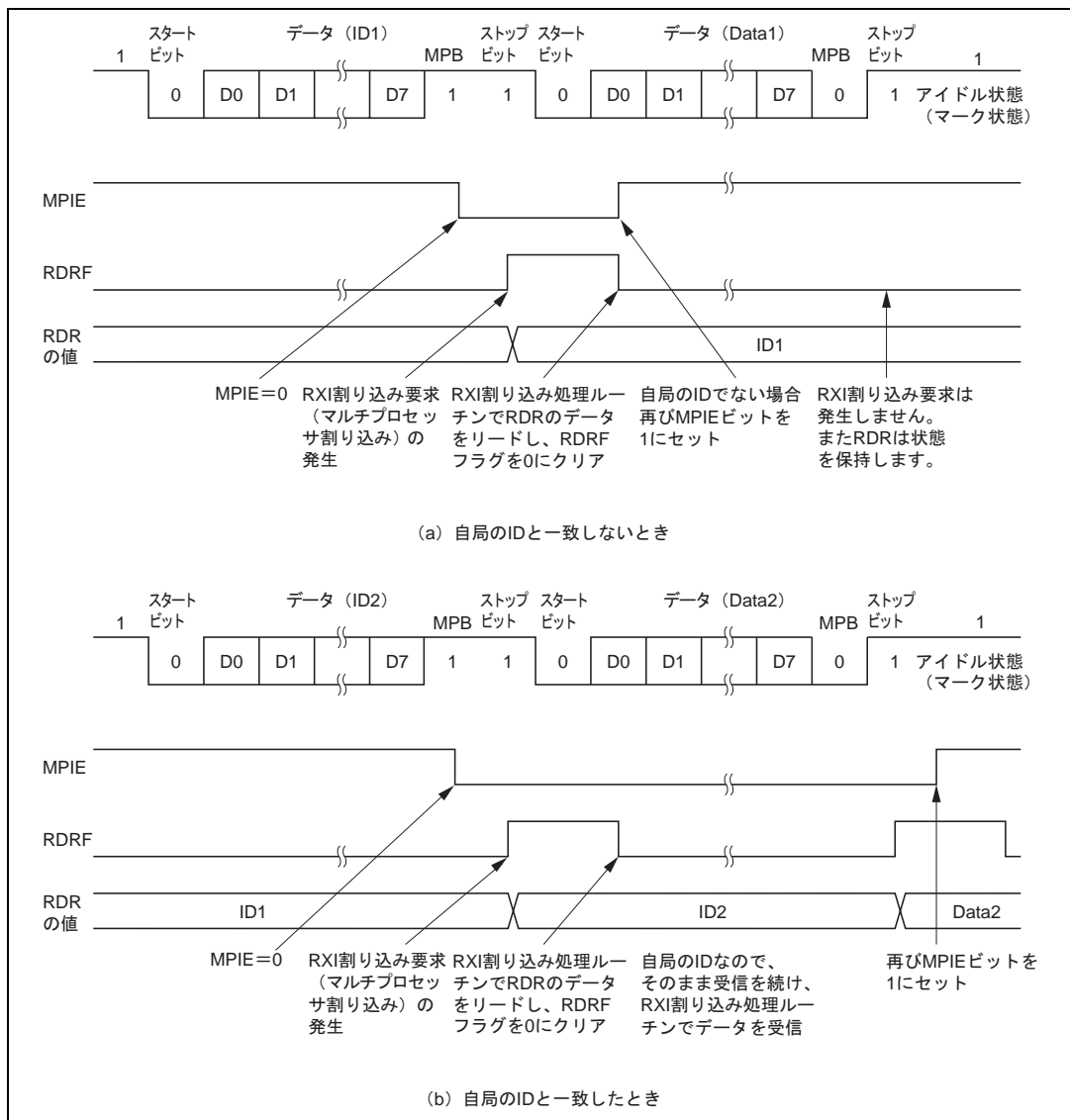
図 14.13 SCI の受信時の動作例 (8ビットデータ/マルチプロセッサビットあり/1ストップビットの例)
