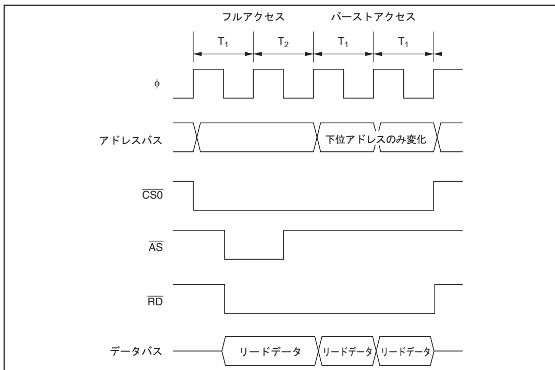
図 6.30 (b) バースト ROM アクセスタイミング例 (AST0 = BRSTS1 = 0 の場合)
