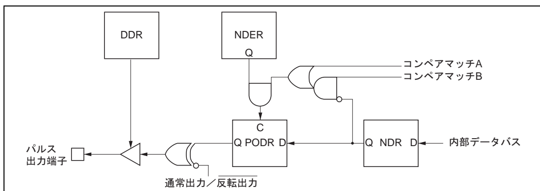
図 11.10 パルス出力ノンオーバーラップ動作
