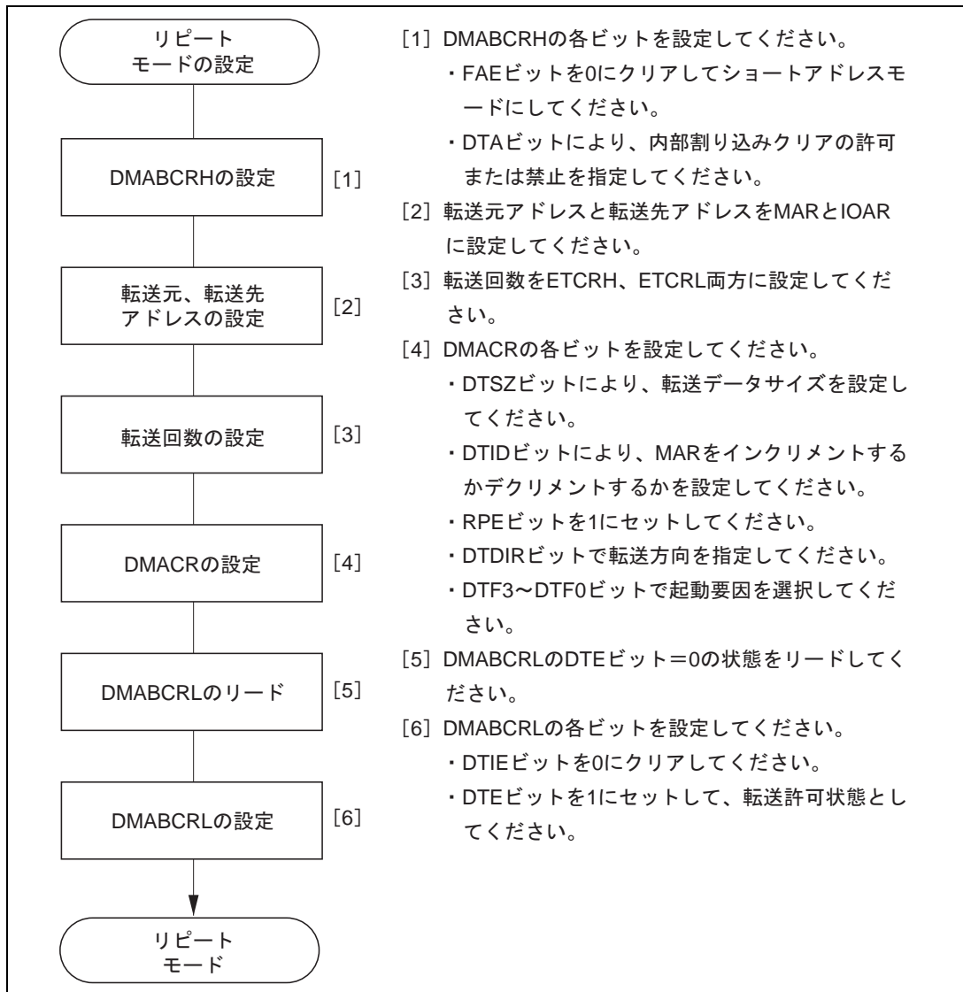
図 7.8 リピートモードの設定手順例
