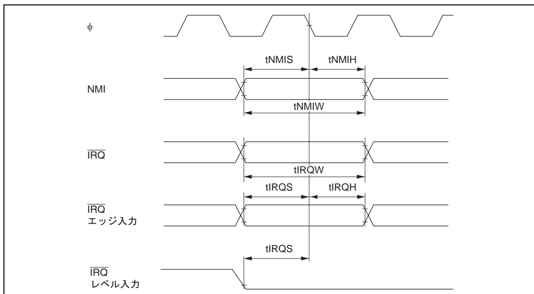
図 22.5 割り込み入力タイミング
