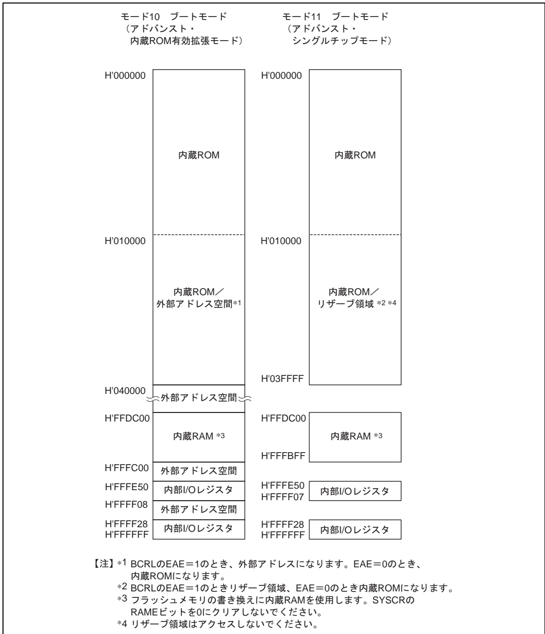
図 3.2 H8S/2328 の各動作モードのアドレスマップ (2) [ F-ZTAT 版のみ ]
