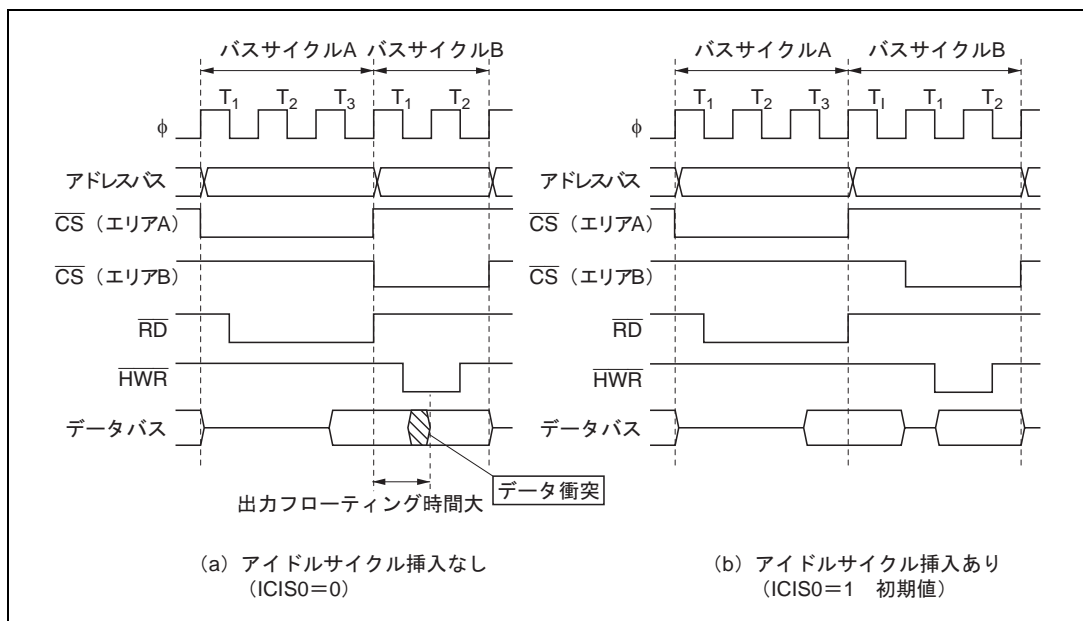
図 6.32 アイドルサイクル動作例 (2)
