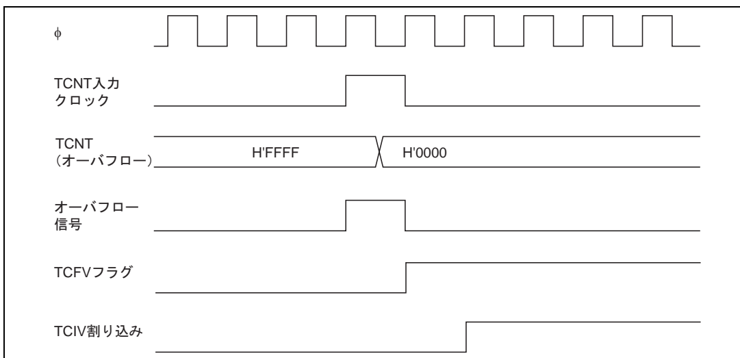
図 10.44 TCIV 割り込みのセットタイミング
