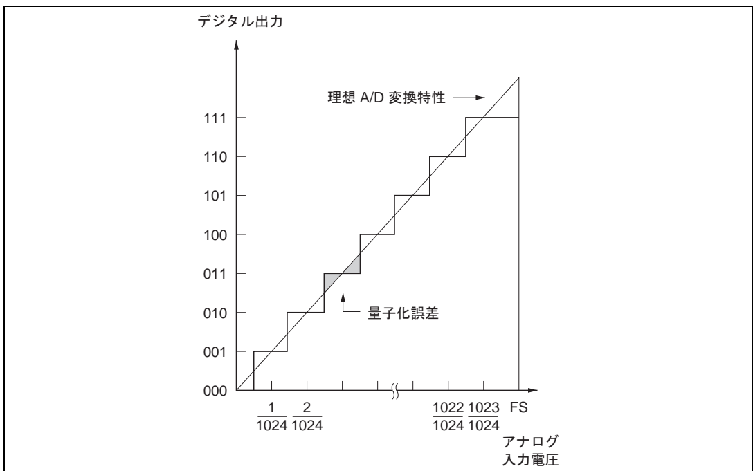
図 16.8 A/D 変換精度の定義 (1)
