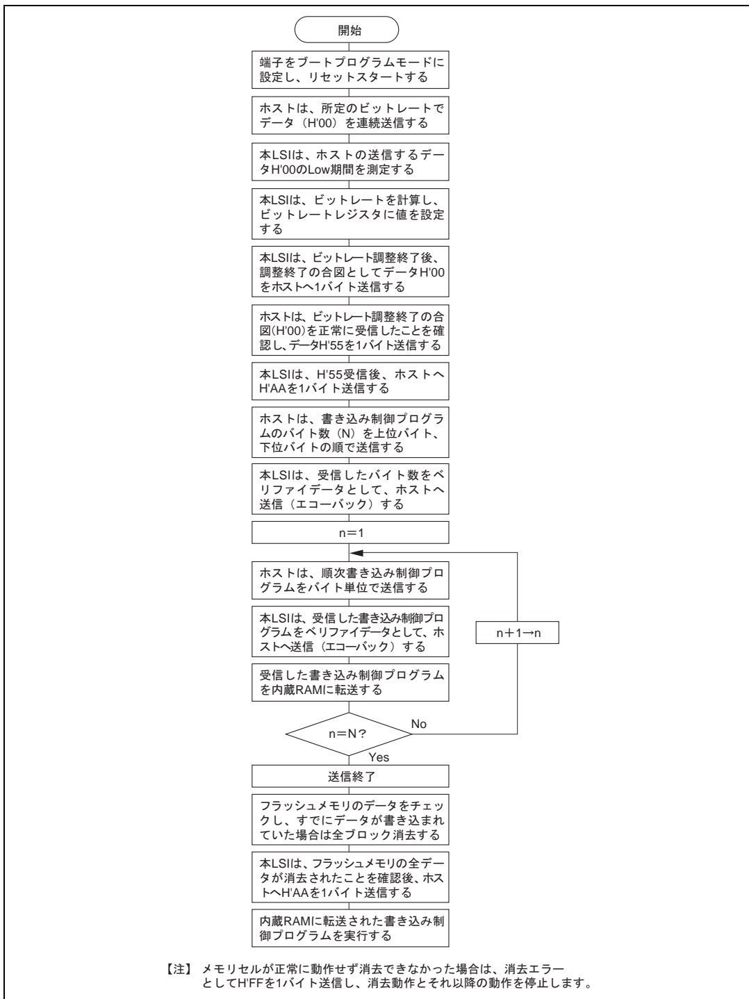
図 19.67 ブートモード実行手順
