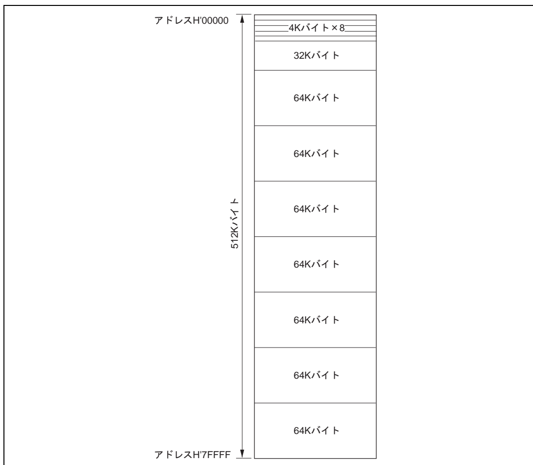
図 19.65 ブロック分割法
