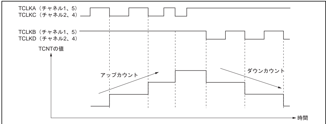
図 10.31 位相計数モード 3 の動作例
