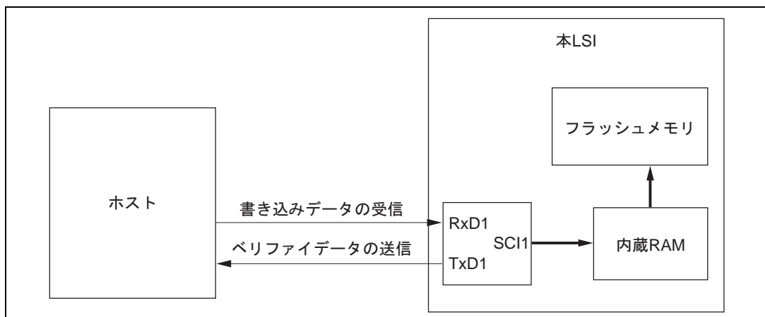
図 19.36 ブートモード時のシステム構成図
