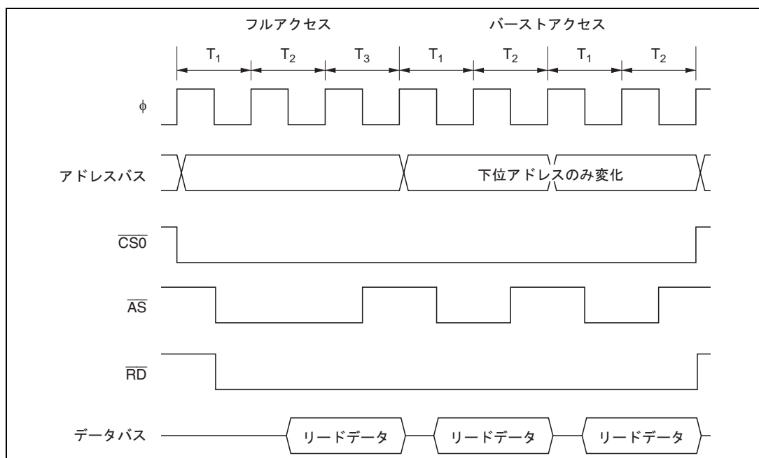
図 6.30 (a) バースト ROM アクセスタイミング例 (AST0 = BRSTS1 = 1 の場合)
