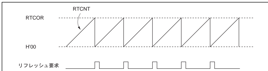
図 6.23 RTCNT の動作
