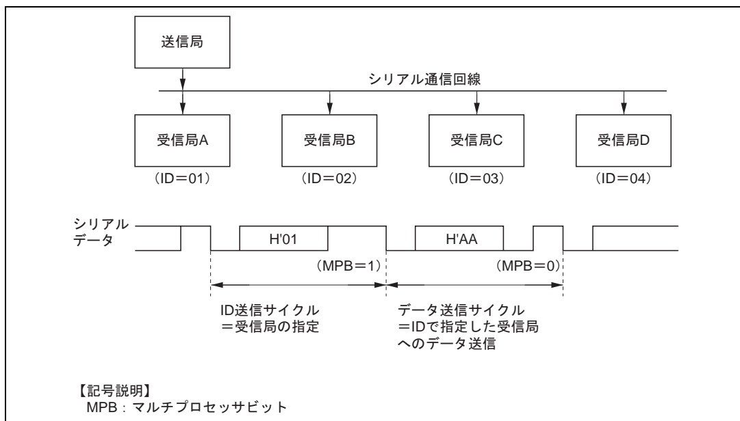
図 14.9 マルチプロセッサフォーマットを使用したプロセッサ間通信の例 (受信局 A へのデータ H'AA の送信の例)
