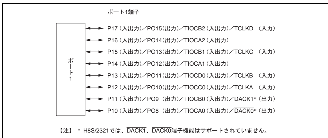
図 9.1 ポート 1 の端子機能
