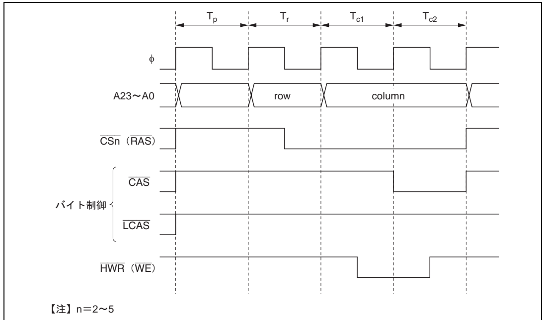
図 6.18 CAS2 本方式の制御タイミング (上位バイトライトアクセス時)
