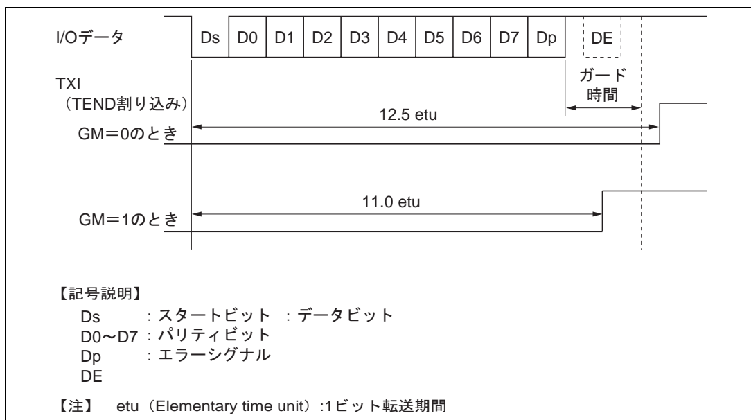
図 15.6 送信動作時の TEND フラグ発生タイミング
