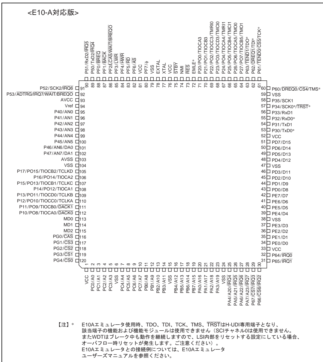
図 1.9 HD64F2329E ピン配置図 (TFP-120 : 上面図)
