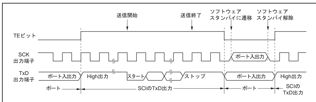
図 14.24 内部クロック、調歩同期送信の場合
