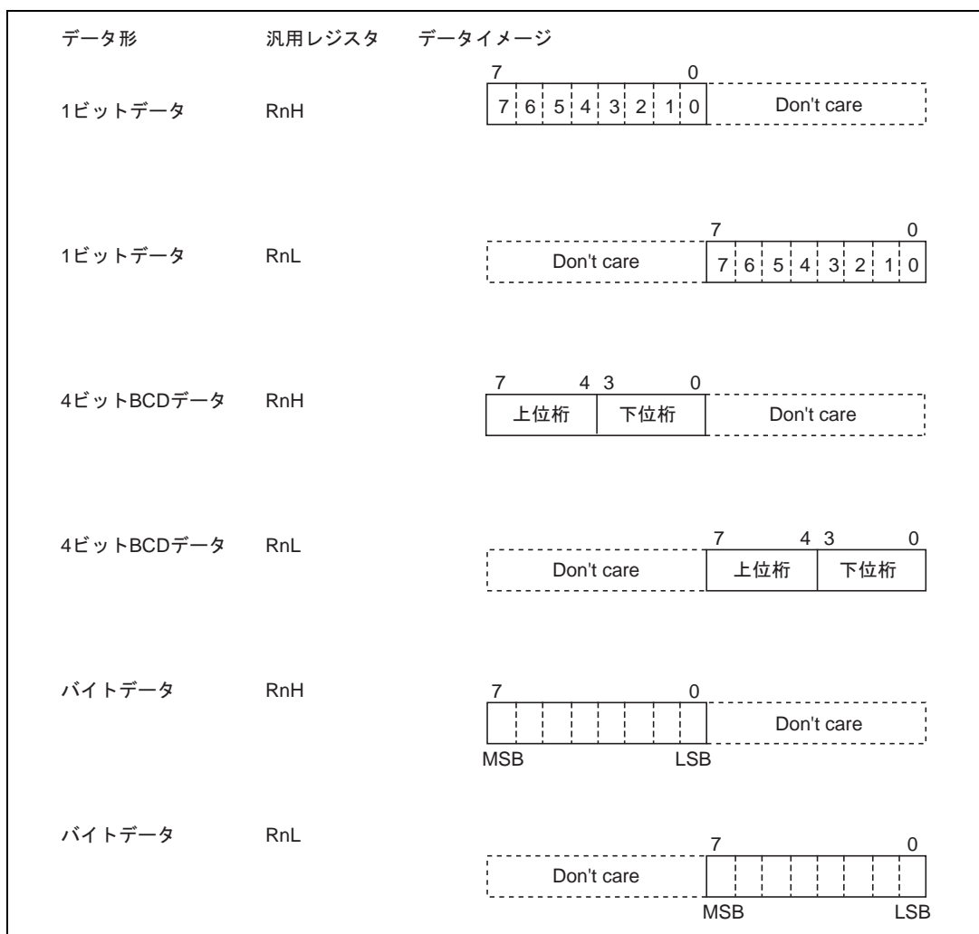
図 2.7 汎用レジスタのデータ構成 (1)
