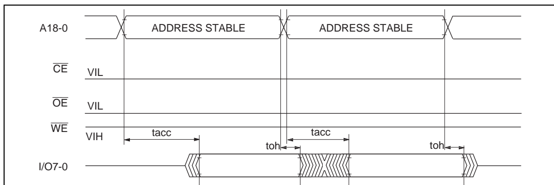
図 19.50 CE、OE イネーブル状態リード時のタイミング波形
