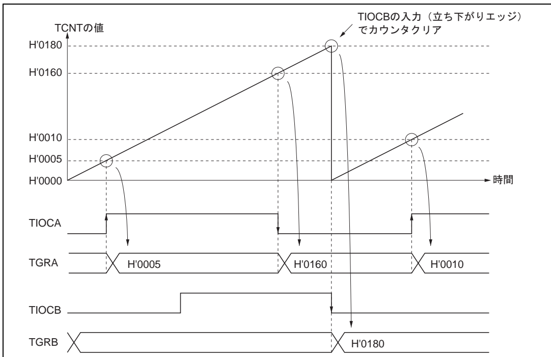
図 10.13 インพุットキャプチャ動作例
