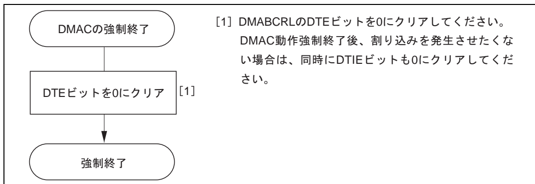
図 7.37 DMAC 動作の強制終了手順例
