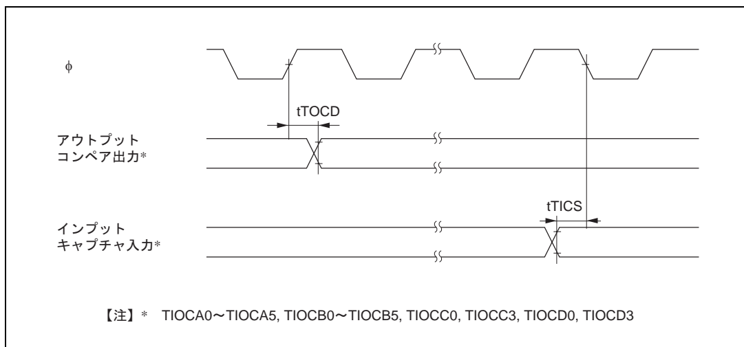
図 22.22 TPU 入出力タイミング
