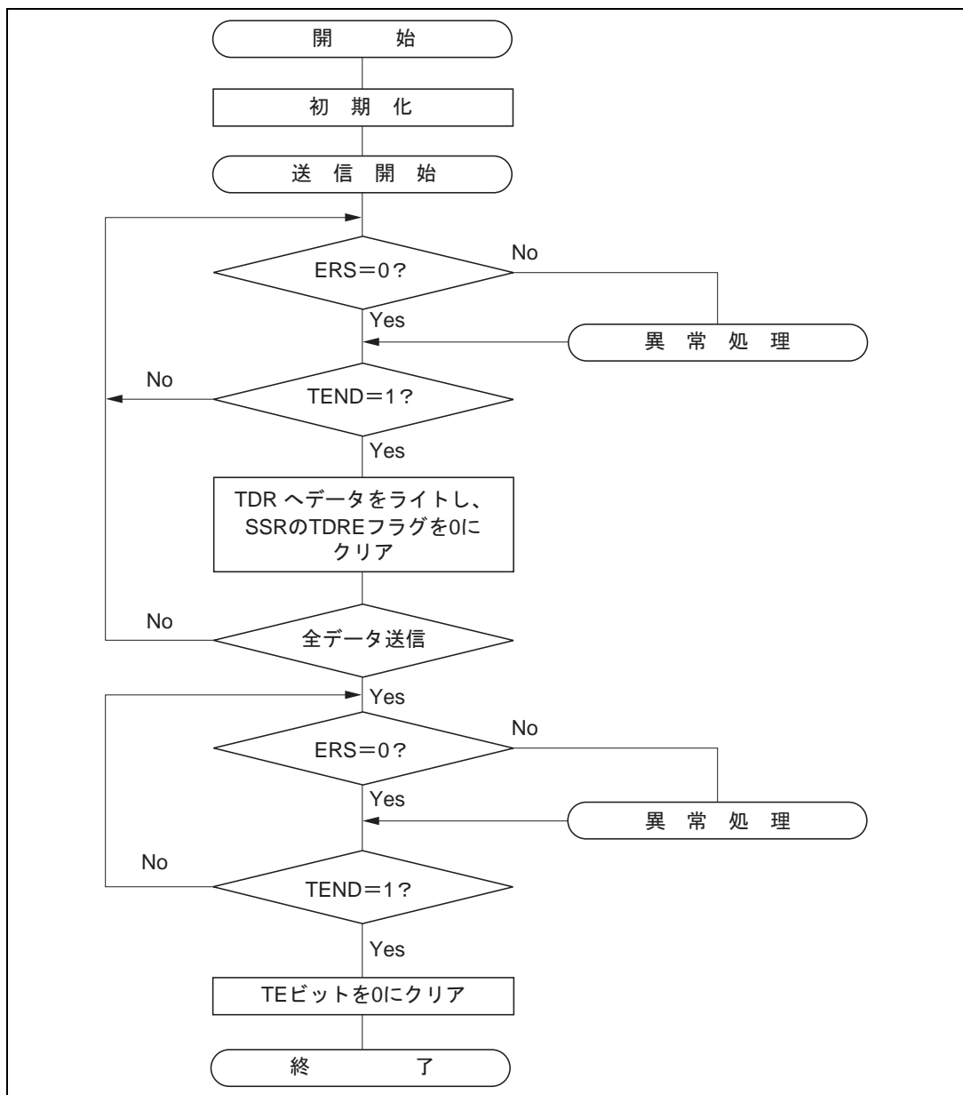
図 15.4 送信処理フローの例
