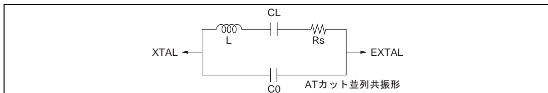
図 20.3 水晶発振子の等価回路
