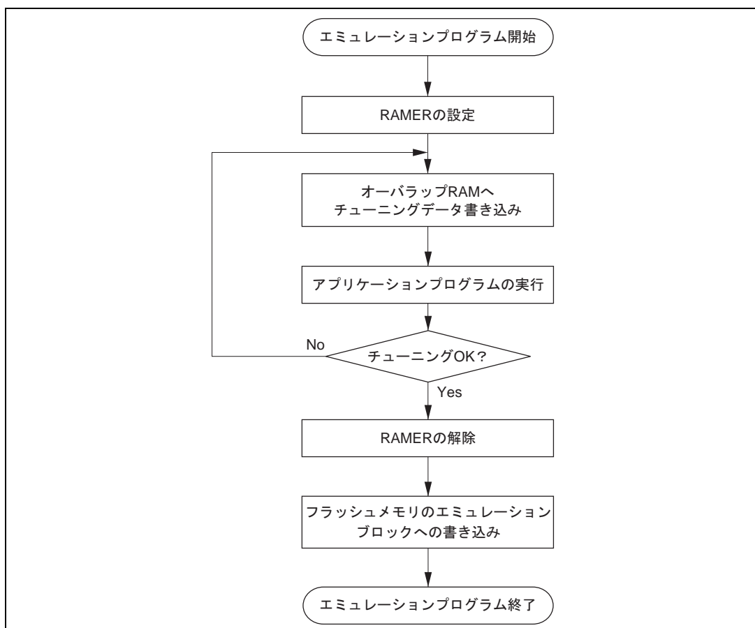
図 19.44 RAM によるエミュレーションフロー
