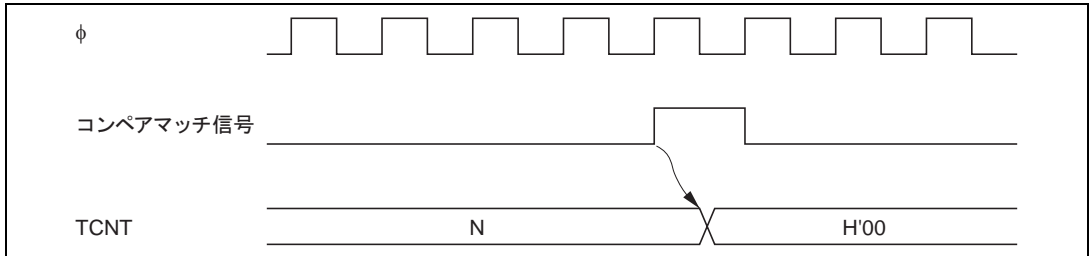
図 12.6 コンペアマッチによるクリアタイミング
