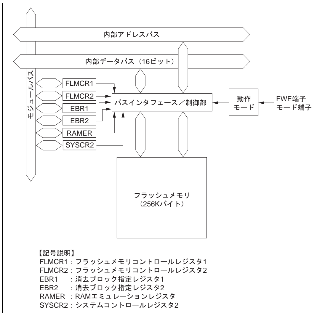
図 19.29 フラッシュメモリのブロック図
