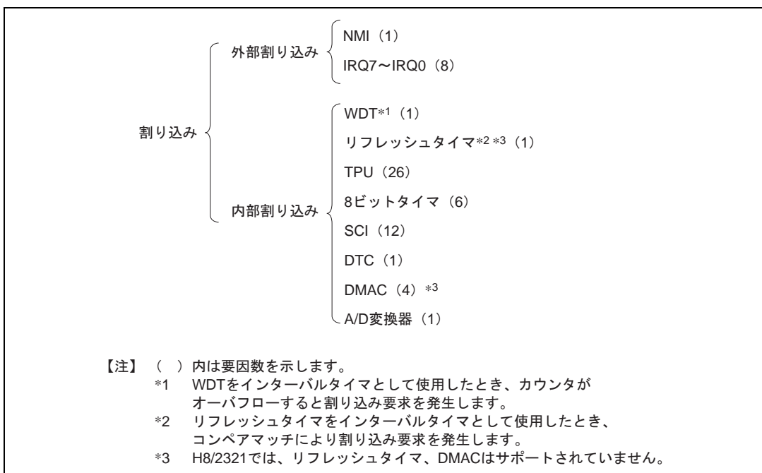
図 4.3 割り込み要因と要因数
