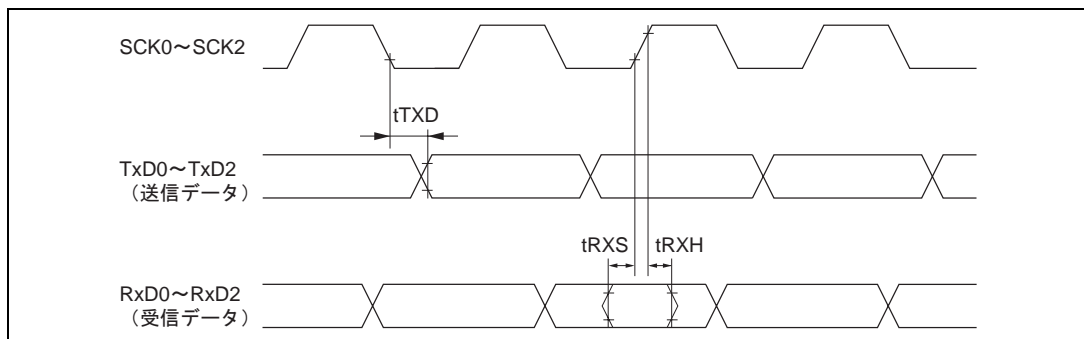
図 22.29 SCI 入出力タイミング/クロック同期式モード
