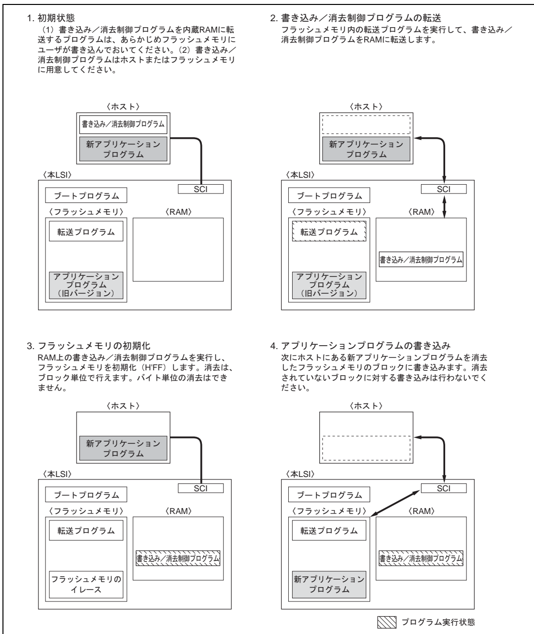
図 19.5 ユーザプログラムモード (例)
