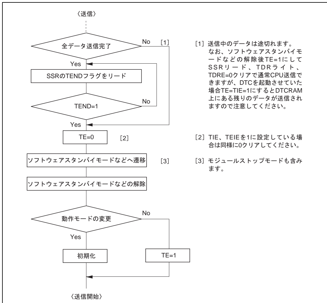
図 14.23 送信時のモード遷移フローチャートの例
