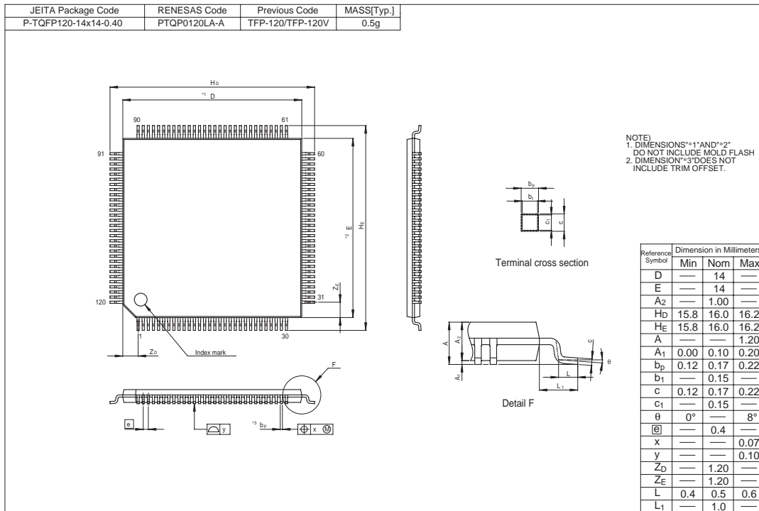
図 G.1 TFP-120 外形寸法図
