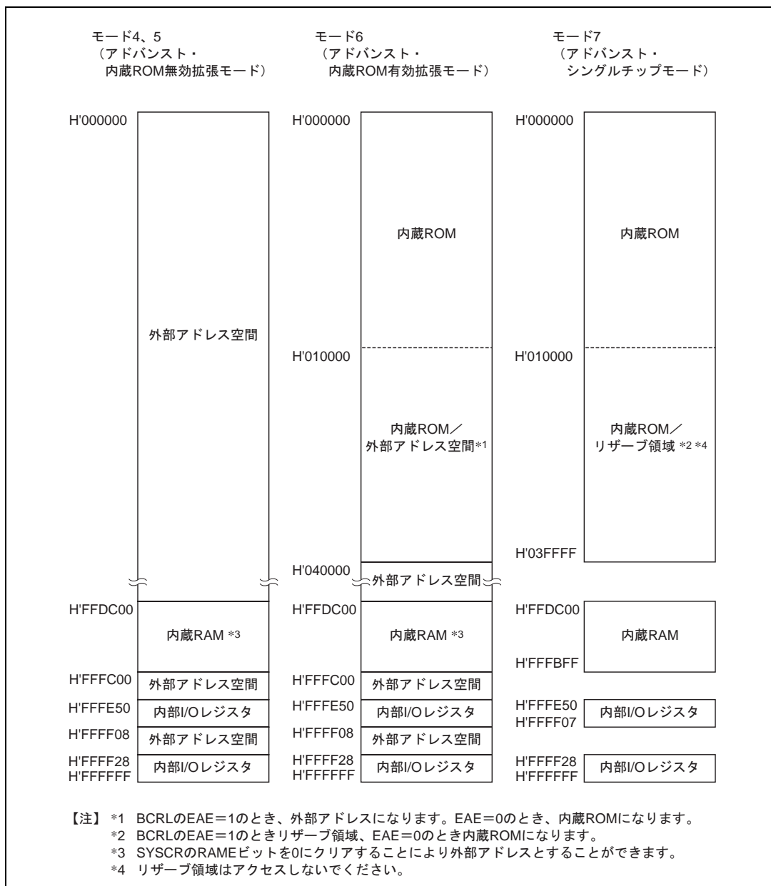
図 3.2 H8S/2328 の各動作モードのアドレスマップ (1)
