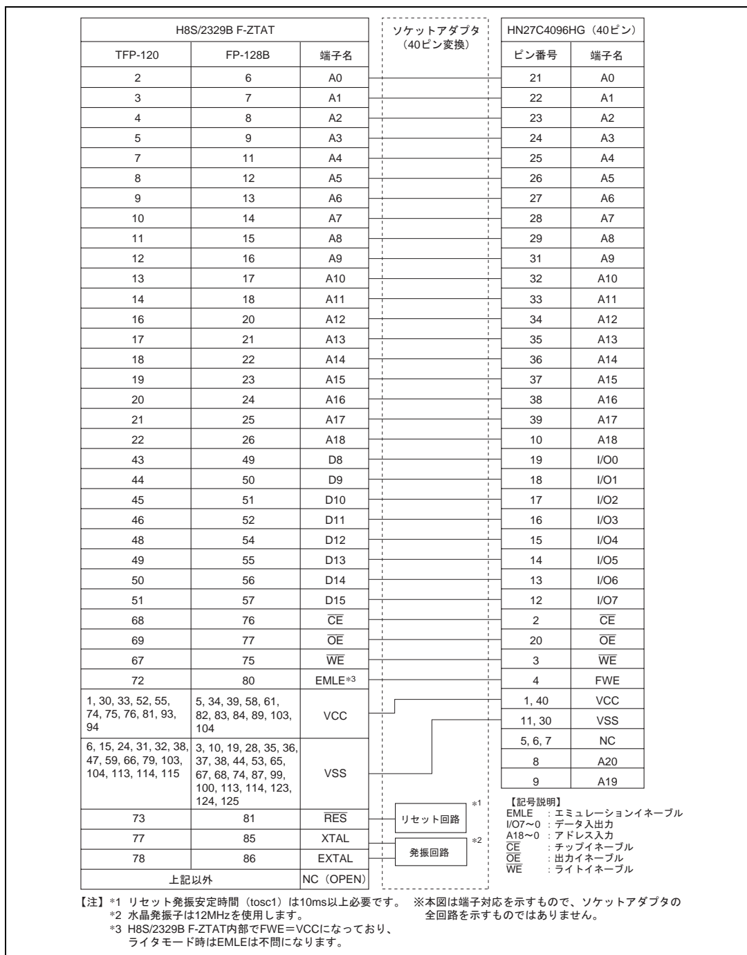
図 19.20 H8S/2329B F-ZTAT ソケットアダプタの端子対応図
