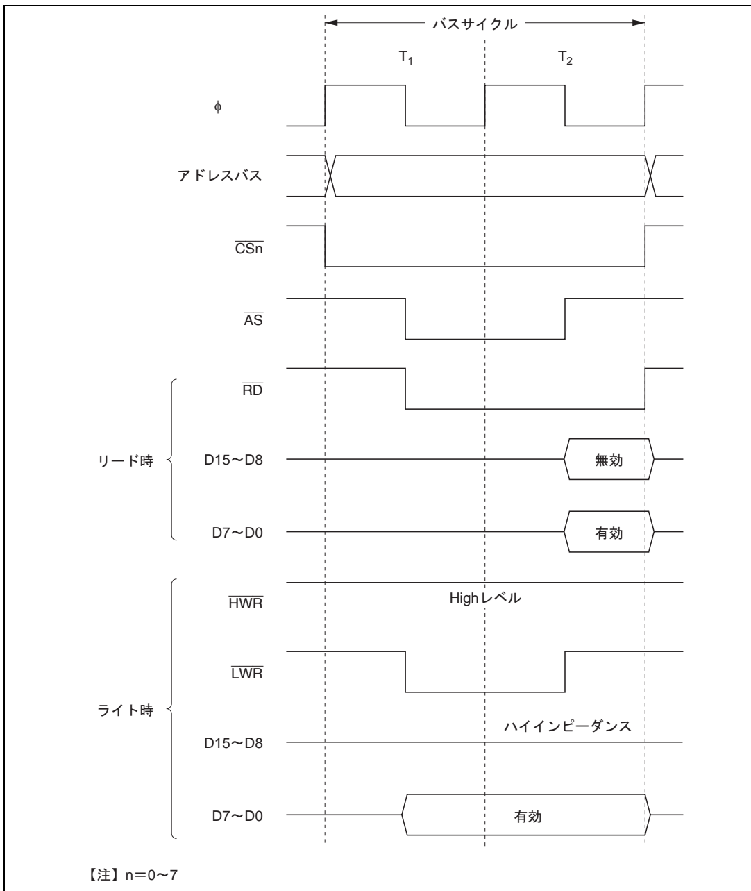
図 6.9 16 ビット 2 ステートアクセス空間のバスタイミング (2) (奇数アドレスバイトアクセス)
