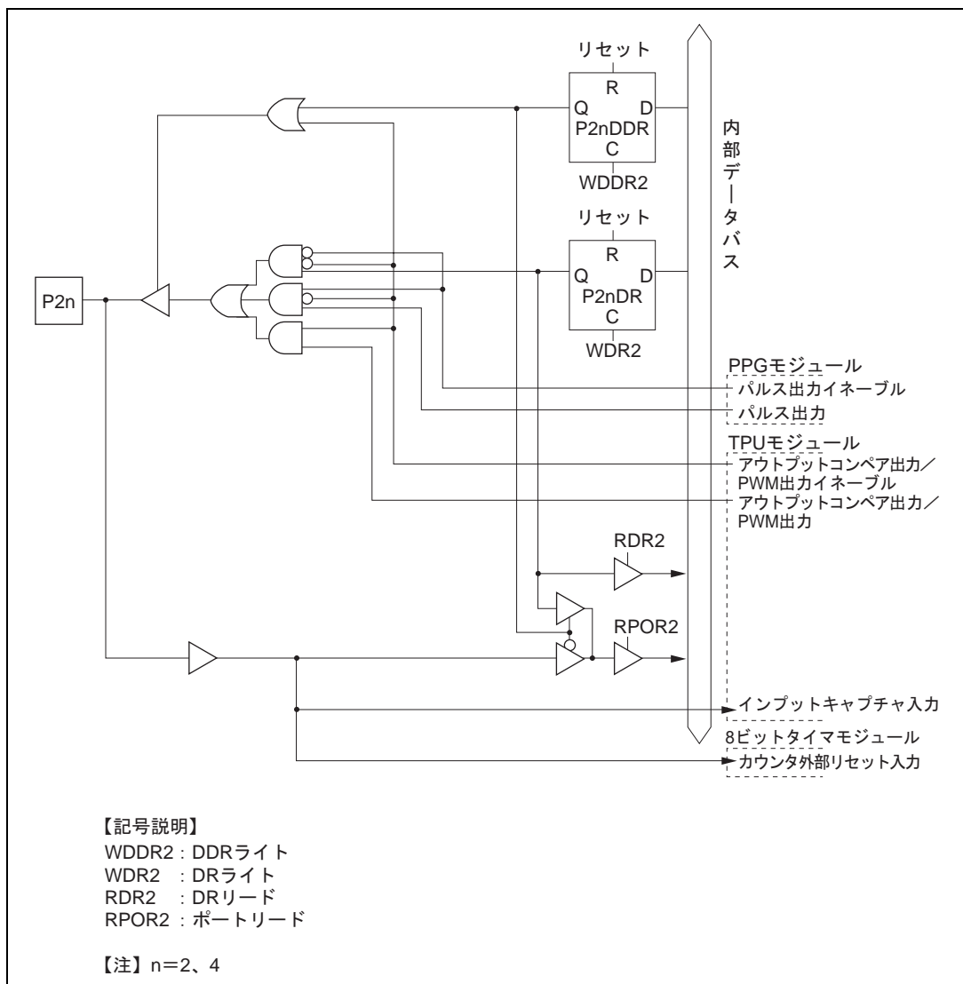
図 C.2 (b) ポート 2 ブロック図 (P22、P24 端子)
