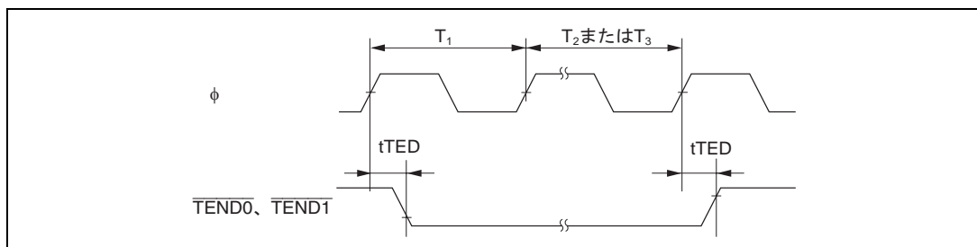
図 22.18 DMAC \overline{TEND} 出カタイミング
