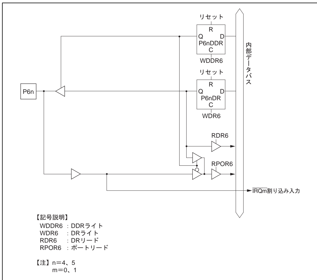
図 C.6 (e) ポート 6 ブロック図 (P64、P65 端子)
