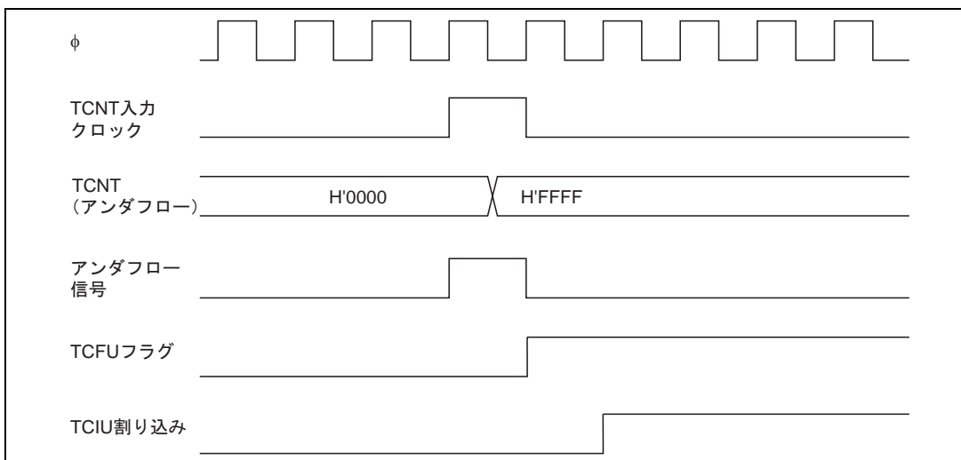
図 10.45 TCIU 割り込みのセットタイミング
