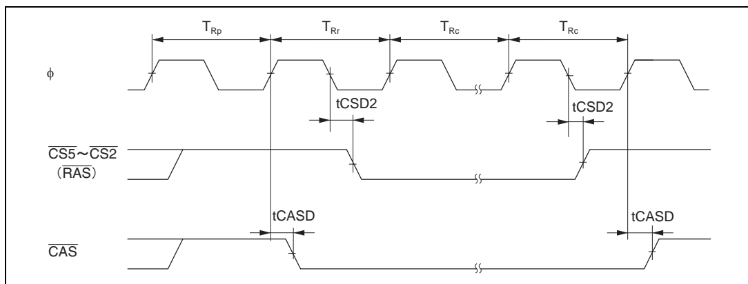
図 22.11 セルフリフレッシュタイミング (H8S/2321 ではサポートされていません)
