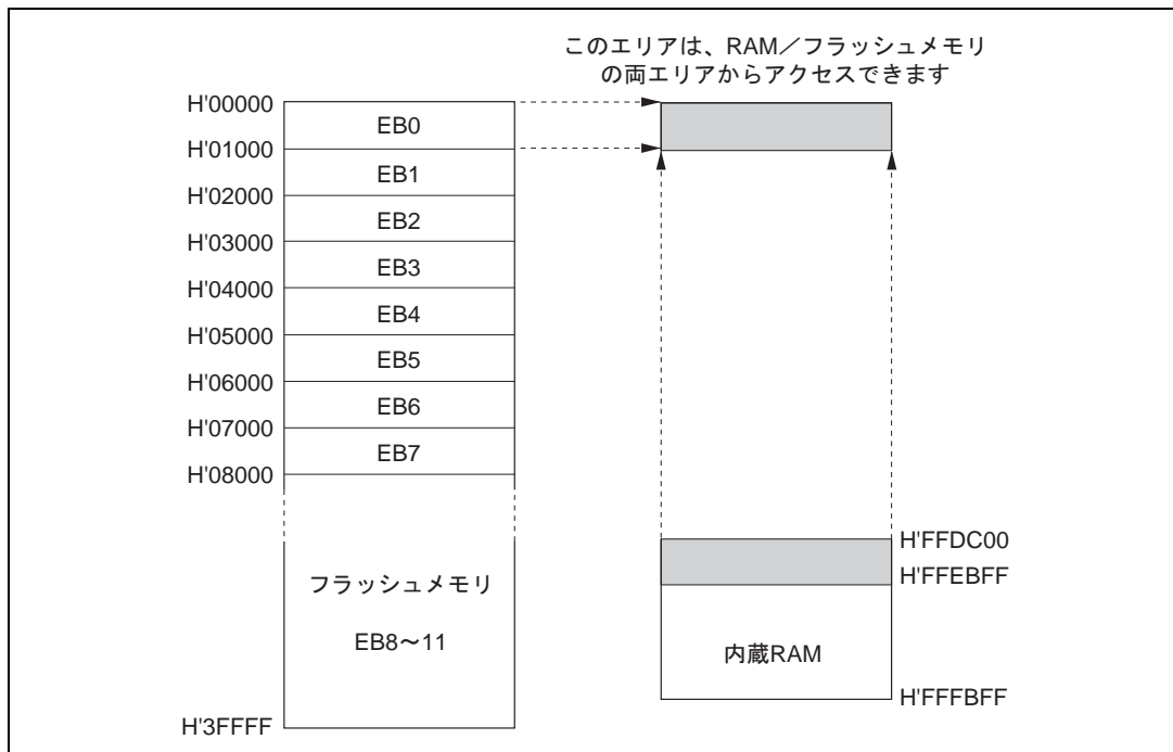
図 19.45 RAM のオーバーラップ動作例
