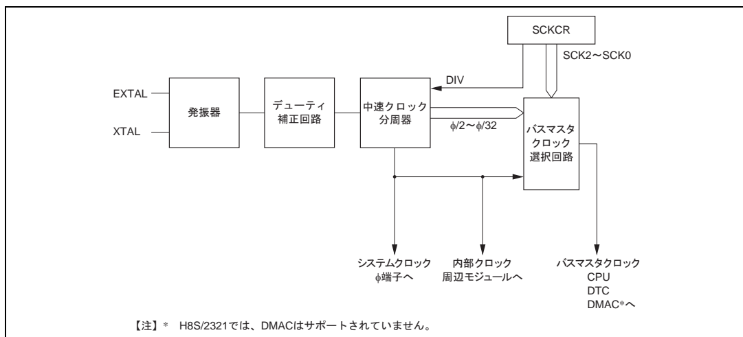
図 20.1 クロック発振器のブロック図
