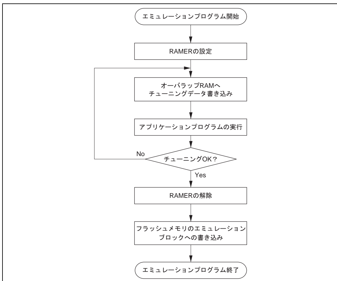
図 19.74 RAM によるエミュレーションフロー
