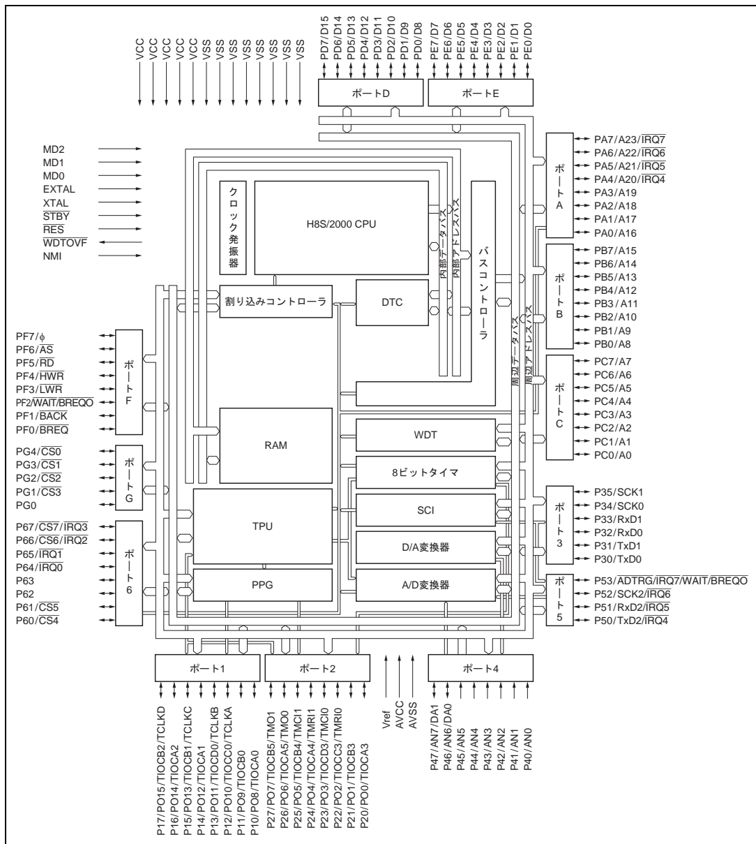
図 1.2 H8S/2321 内部ブロック図
