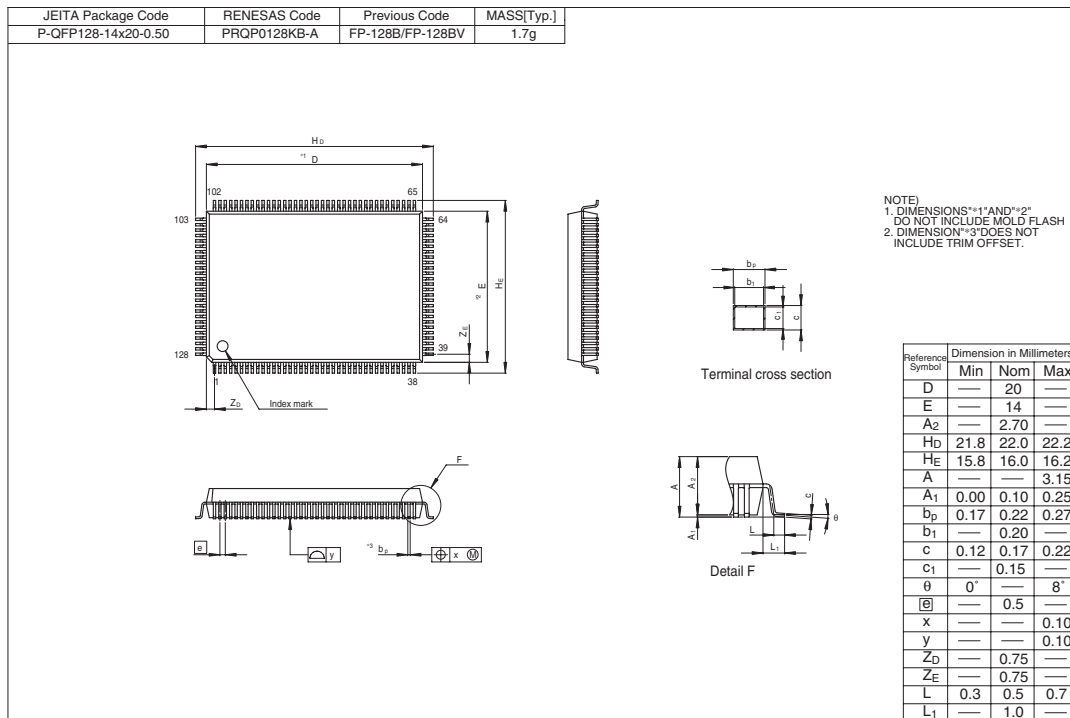
図 G.2 FP-128B 外形寸法図
