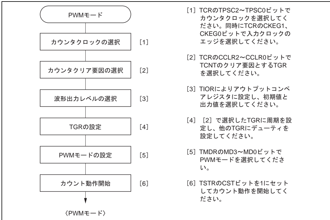
図 10.24 PWMモードの設定手順例
