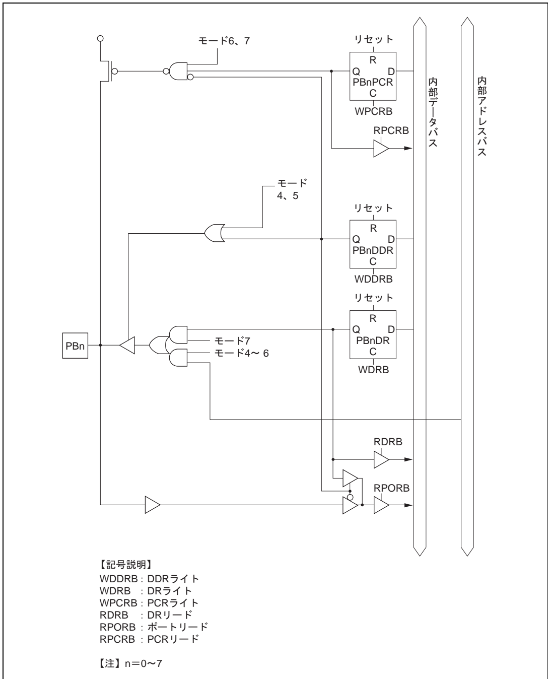
図 C.8 ポート B ブロック図 (PB0~PB7 端子)
