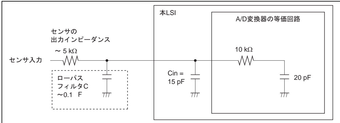
図 16.10 アナログ入力回路の例
