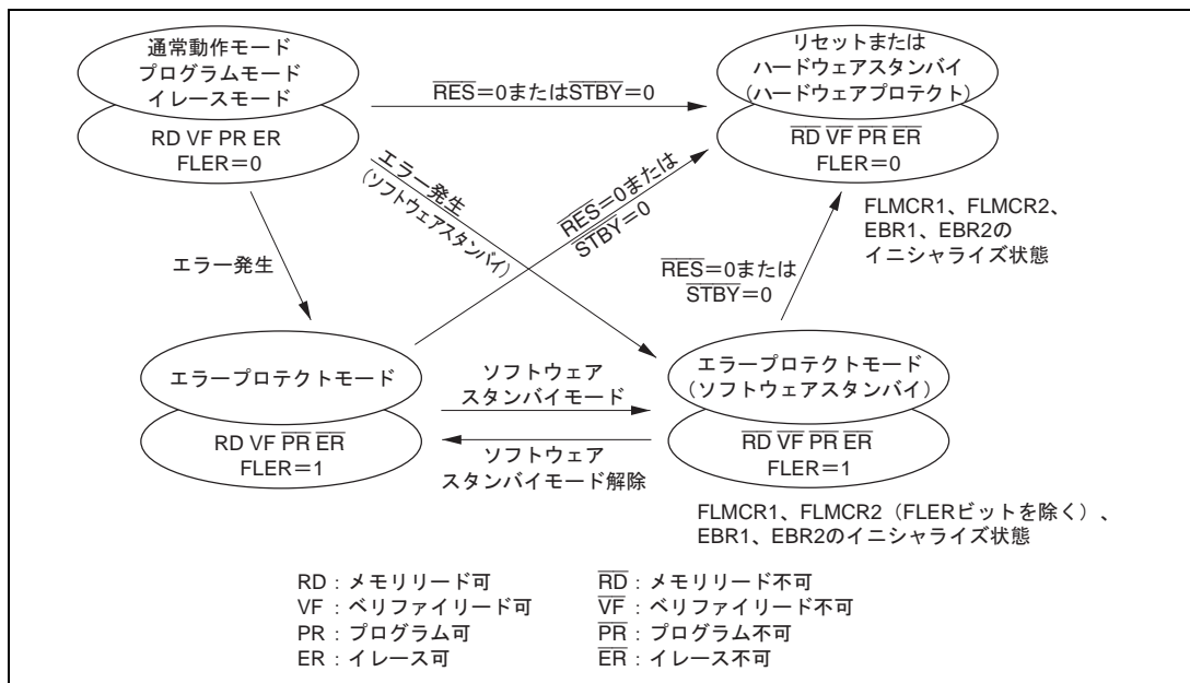
図 19.43 フラッシュメモリの状態遷移図
