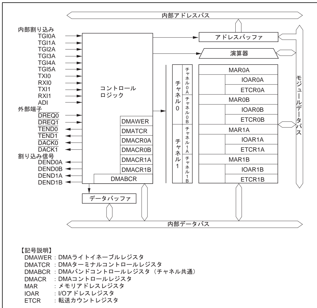
図 7.1 DMAC のブロック図
