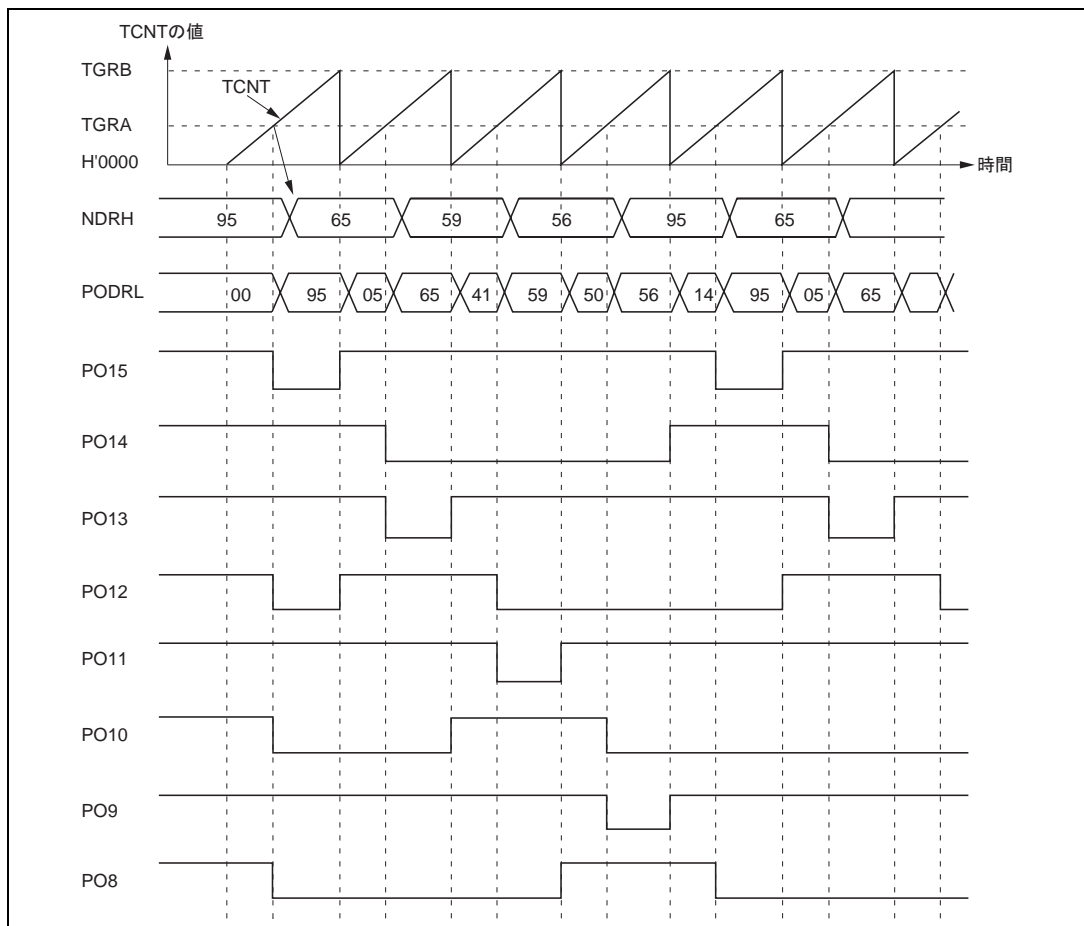
図 11.8 パルス反転出力例
