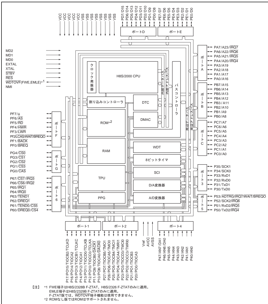
図 1.1 マスク ROM 版、F-ZTAT 版、H8S/2324S、H8S/2322R、H8S/2320 内部ブロック図
