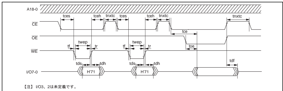
図 19.84 ステータス読み出しモードのタイミング波形
