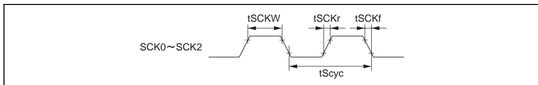
図 22.28 SCK クロック入力タイミング
