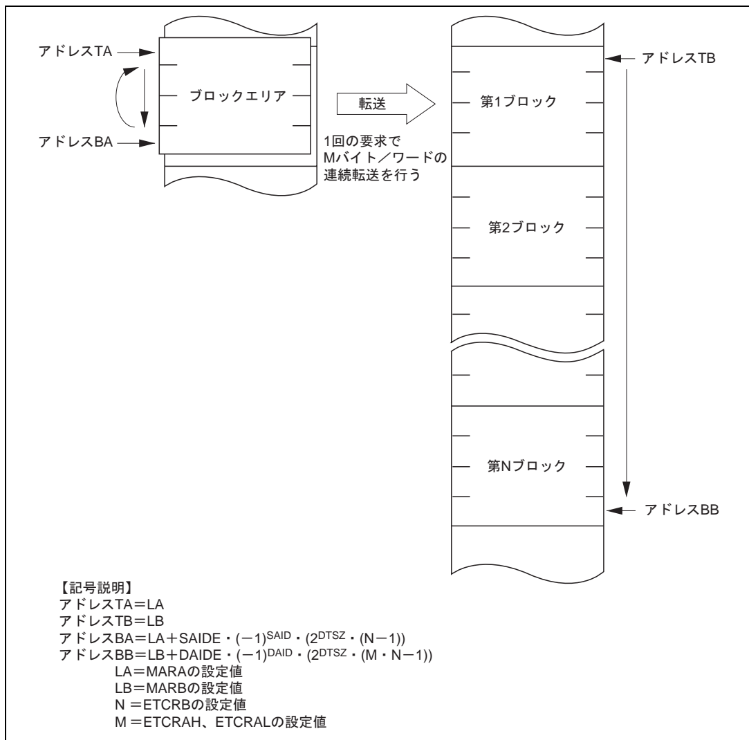
図 7.14 ブロック転送モードの動作 (BLKDIR = 1)
