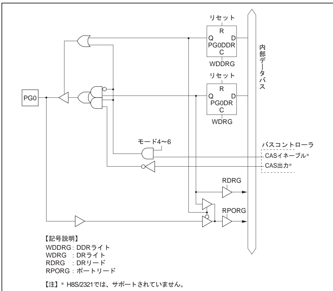
図 C.13 (a) ポート G ブロック図 (PG0 端子)
