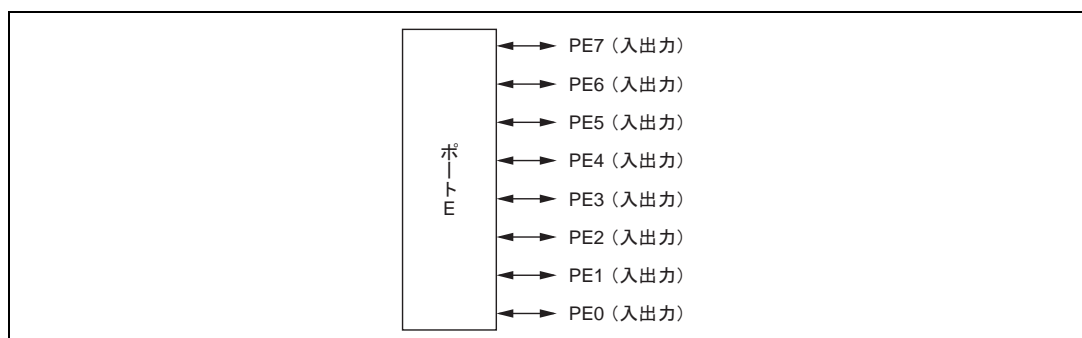
図 9.21 ポート E の端子機能 (モード 7)
