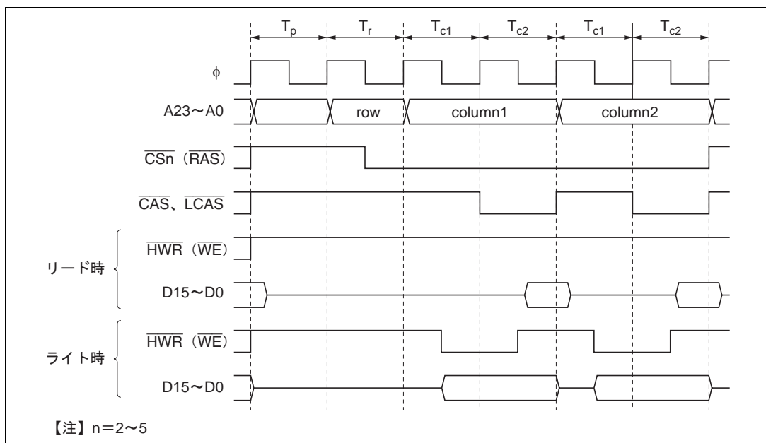
図 6.20 高速ページモードの動作タイミング
