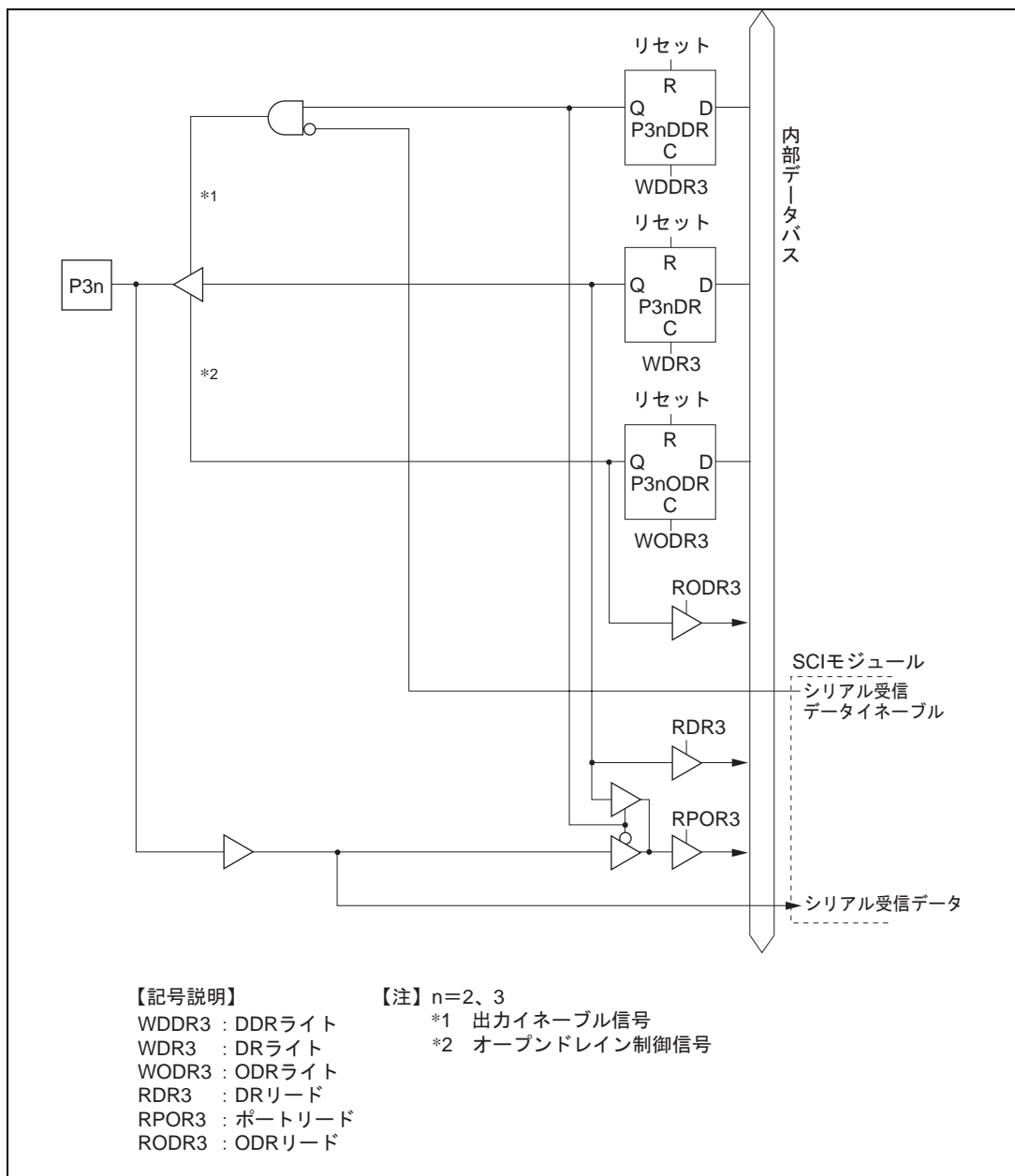
図 C.3 (b) ポート 3 ブロック図 (P32、P33 端子)
