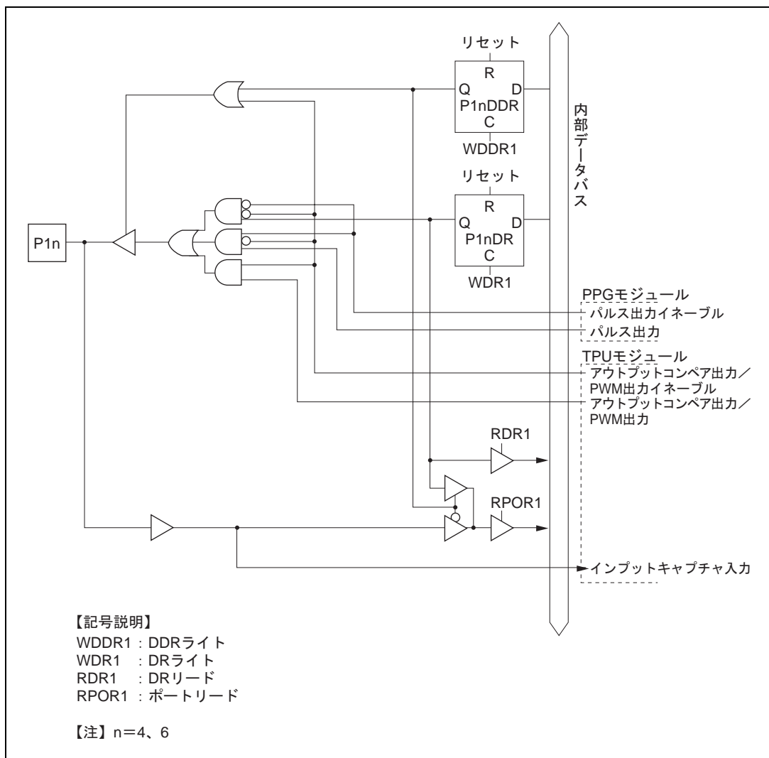
図 C.1 (c) ポート 1 ブロック図 (P14、P16 端子)
