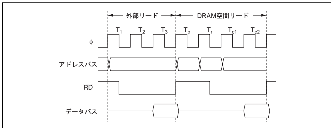
図 6.34 外部リード後の DRAM アクセス例
