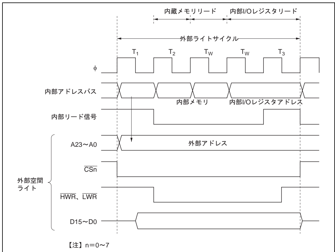
図 6.36 ライトデータバッファ機能使用時のタイミング例
