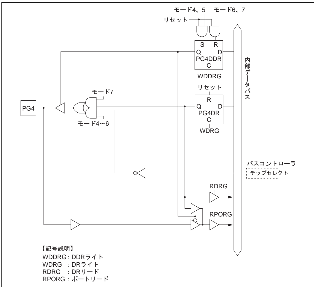
図 C.13 (d) ポート G ブロック図 (PG4 端子)
