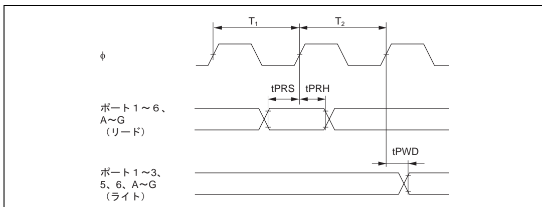
図 22.20 I/O ポート入出力タイミング
