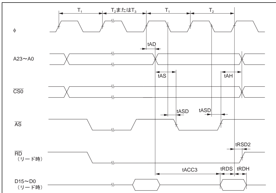
図 22.12 バーストROMアクセスタイミング / 2 ステートアクセス
