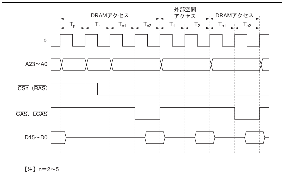
図 6.21 RAS ダウンモードの動作タイミング例
