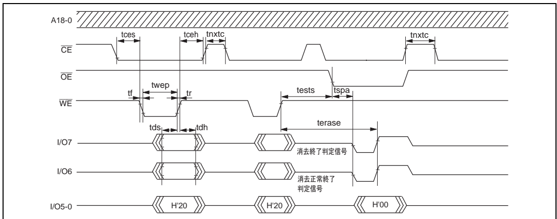
図 19.26 自動消去モードのタイミング波形
