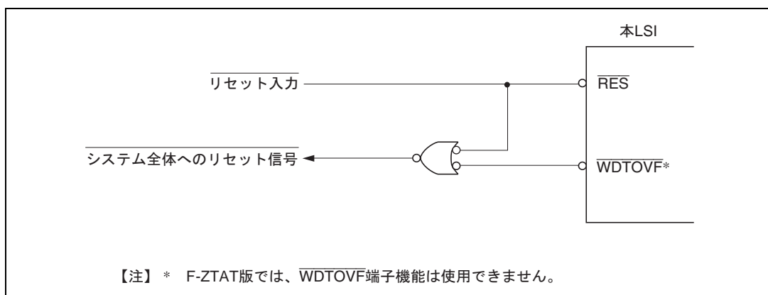
図 13.9 \overline{\text{WDTOVF}} 信号によるシステムのリセット回路例
