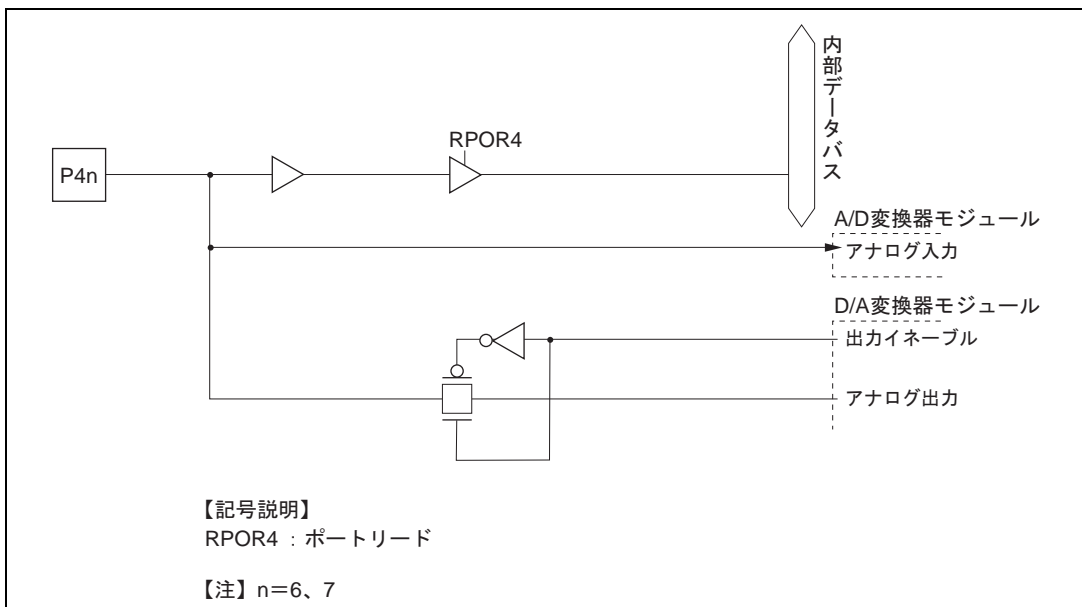
図 C.4 (b) ポート 4 ブロック図 (P46、P47 端子)
