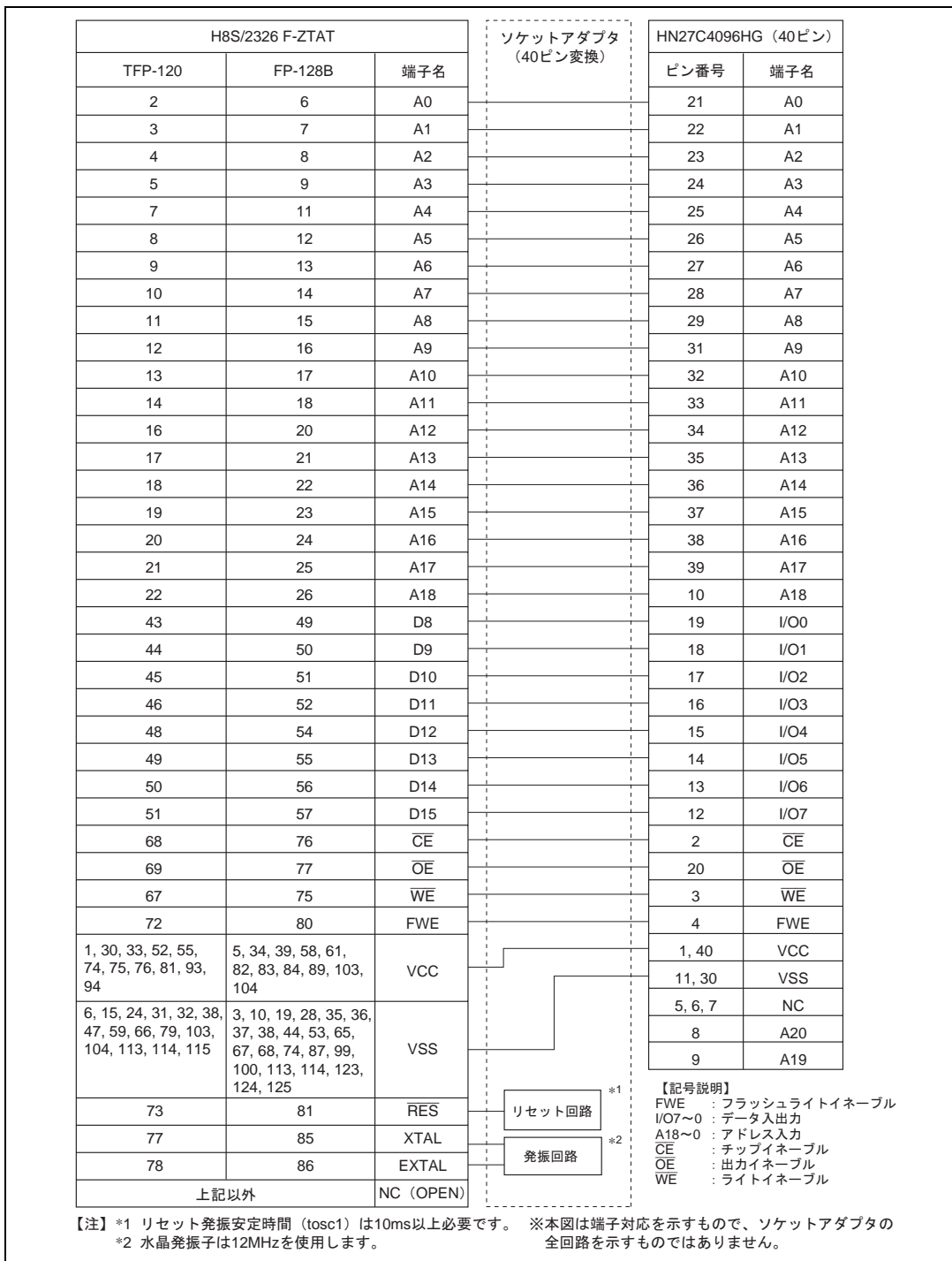
図 19.77 H8S/2326 F-ZTAT ソケットアダプタの端子対応図
