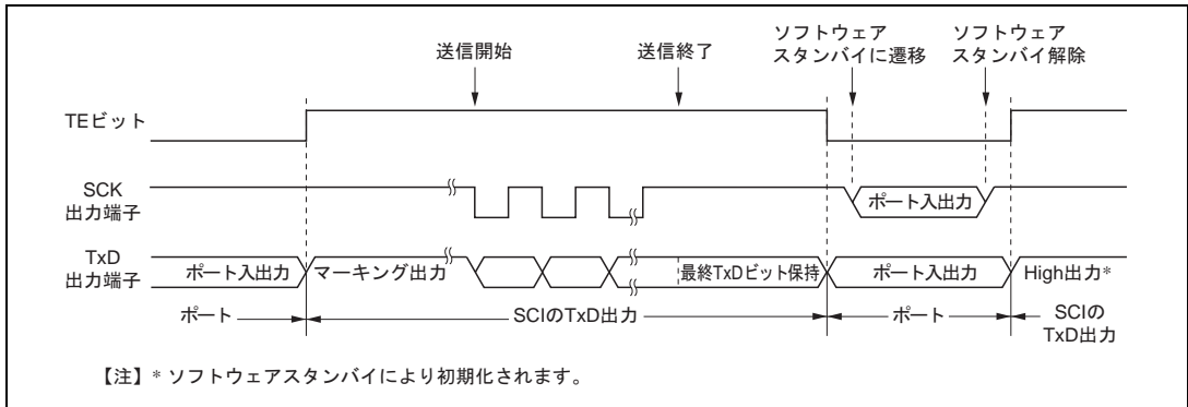
図 14.25 内部クロック、クロック同期送信の場合
