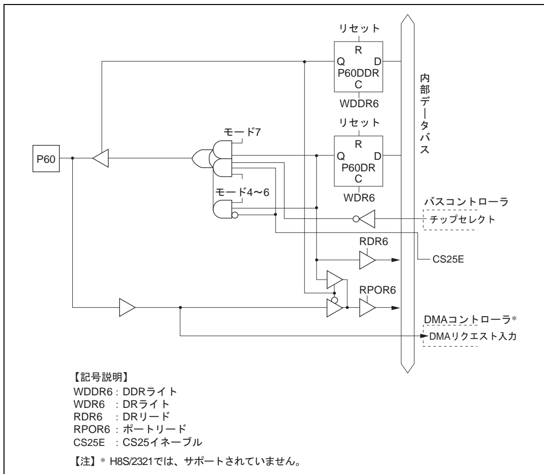
図 C.6 (a) ポート 6 ブロック図 (P60 端子)
