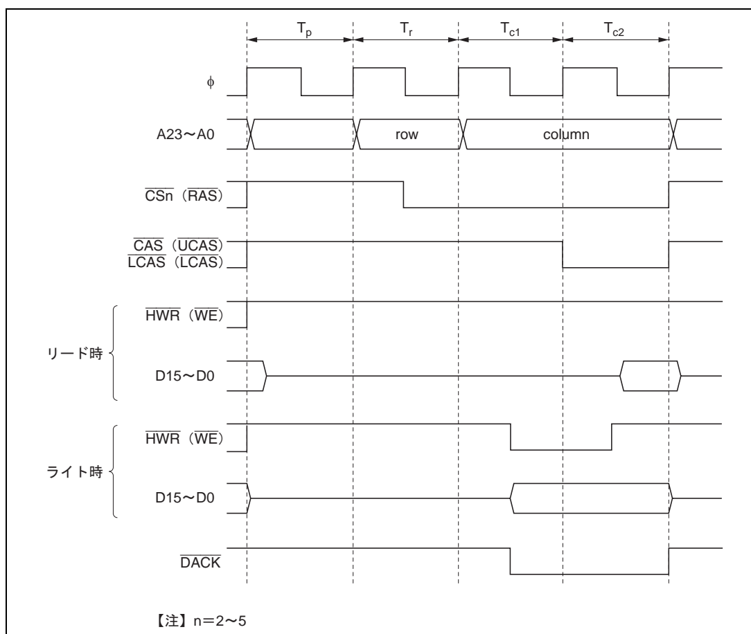
図 6.28 DDS = 1 の場合の \overline{\text{DACK}} 出力タイミング (DRAM アクセスの例)
