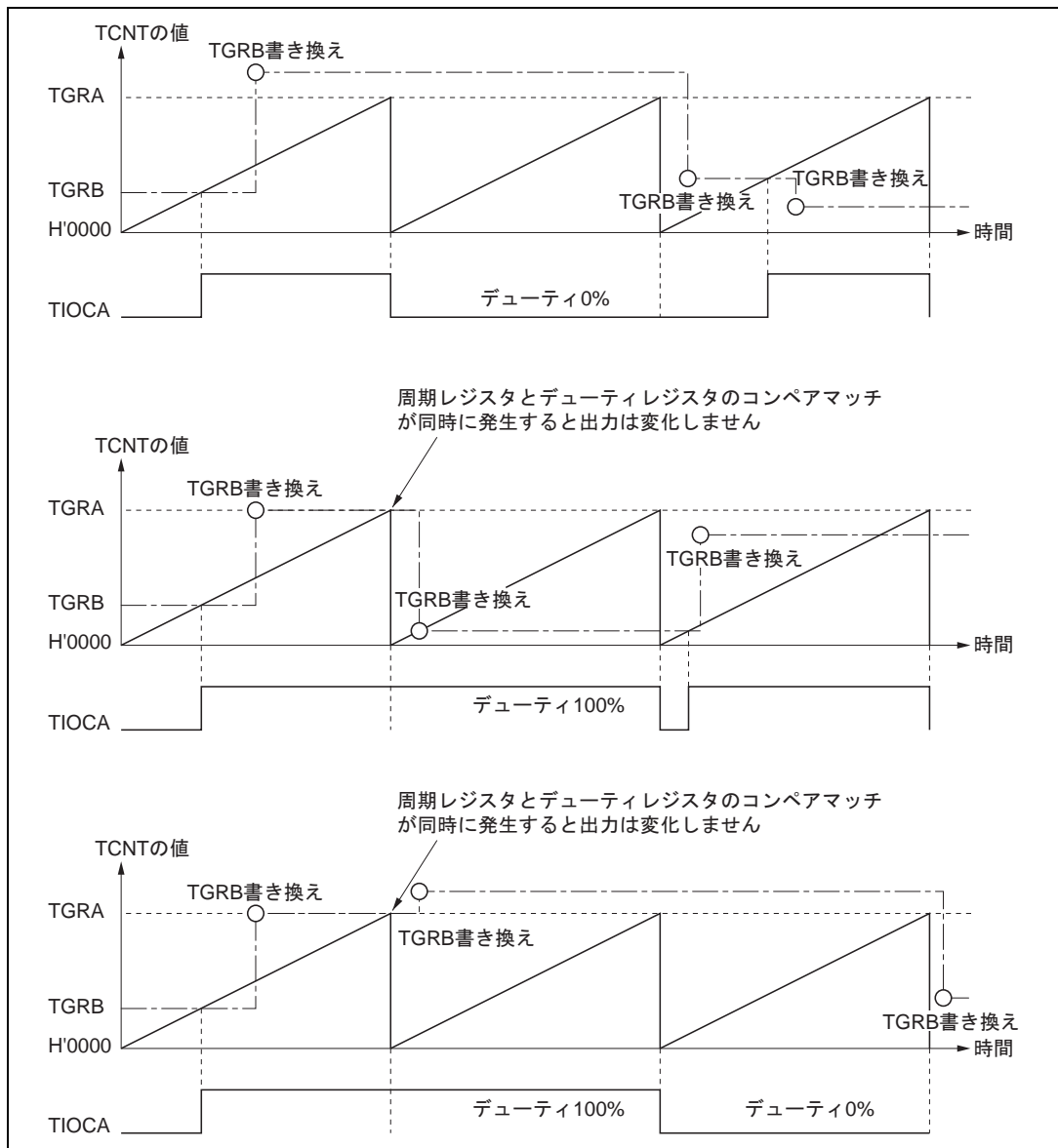
図 10.27 PWM モード動作例 (3)
