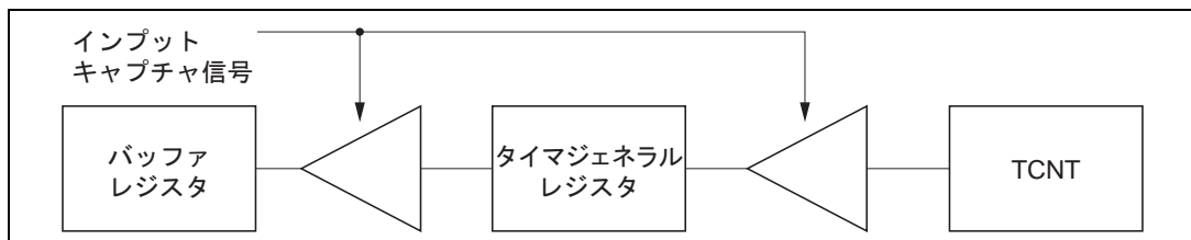
図 10.17 インพุットキャプチャバッファ動作
