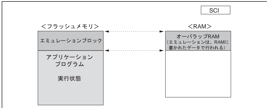
図 19.63 ユーザモード、ユーザプログラムモードのオーバーラップ RAM データの読み出し
