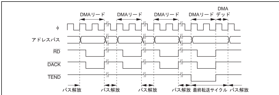
図 7.27 シングルアドレスモード (バイトリード) 転送例
