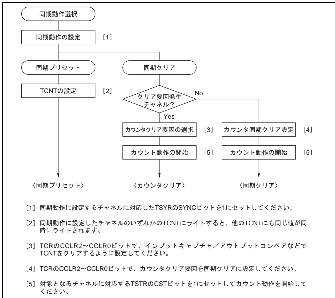
図 10.14 同期動作の設定手順例
