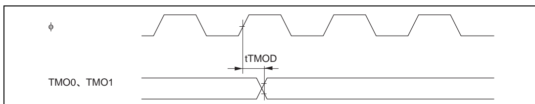
図 22.24 8ビットタイマ出力タイミング
