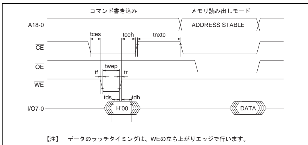
図 19.48 コマンド書き込み後メモリ読み出しタイミング波形
