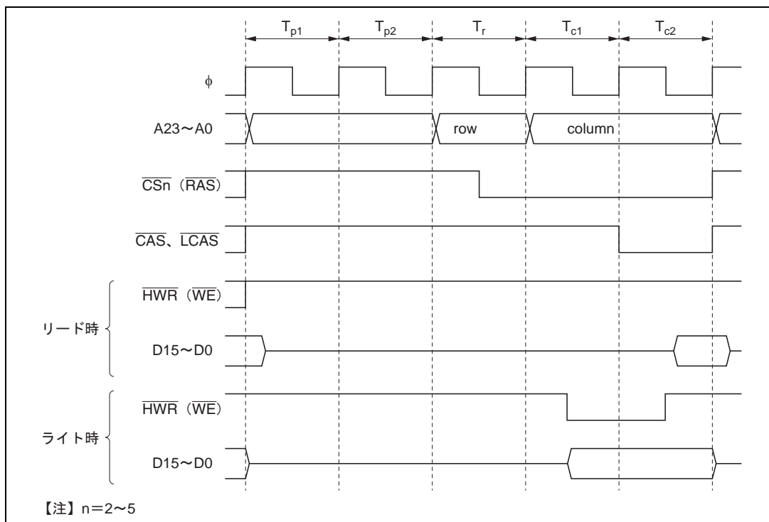
図 6.16 プリチャージサイクル 2 ステート時のタイミング
