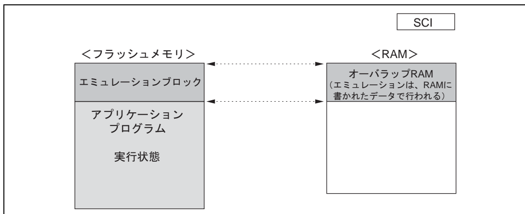
図 19.33 ユーザモード、ユーザプログラムモードのオーバーラップ RAM データの読み出し
