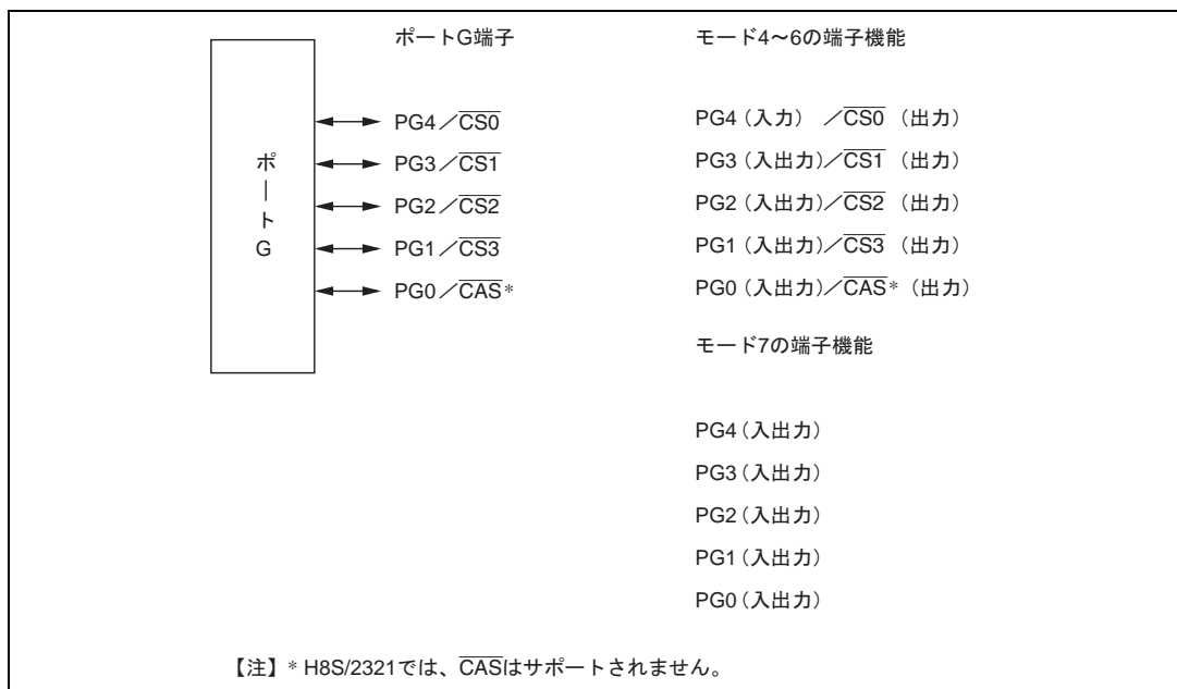
図 9.23 ポート G の端子機能
