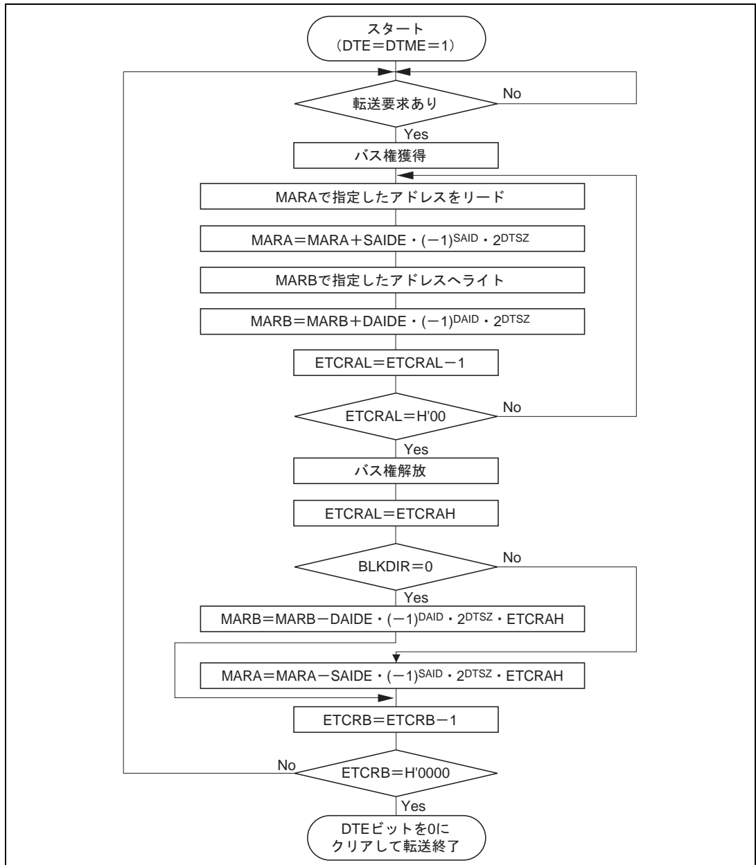
図 7.15 ブロック転送モードの動作フロー
