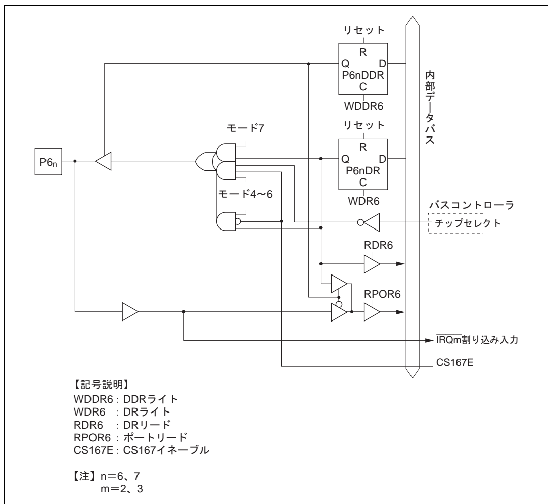
図 C.6 (f) ポート 6 ブロック図 (P66、P67 端子)
