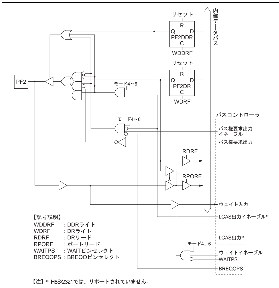
図 C.12 (c) ポート F ブロック図 (PF2 端子)
