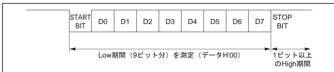
図 19.11 SCI ビットレートの自動合わせ込み動作
