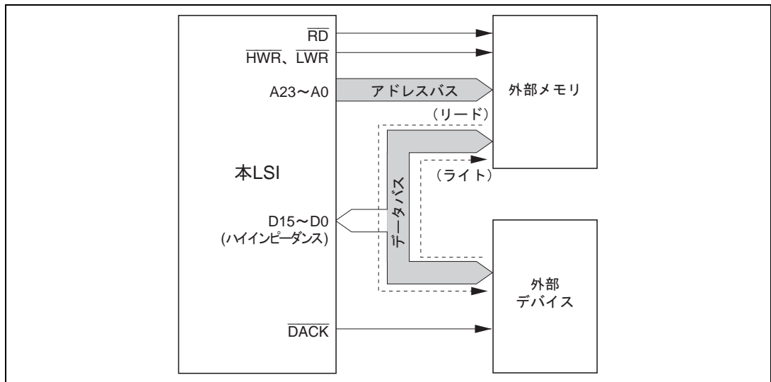
図 7.17 シングルアドレスモード時のデータバス
