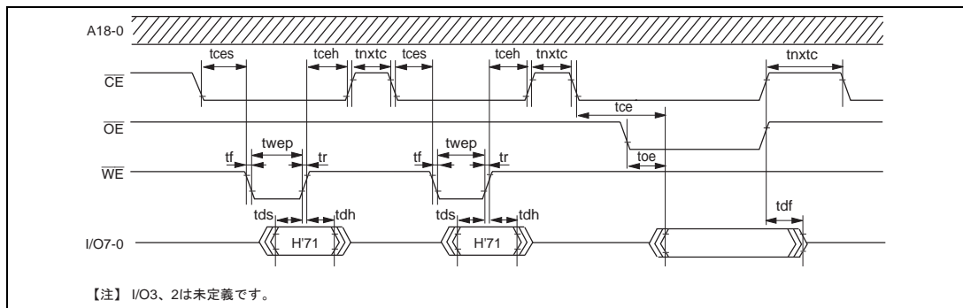
図 19.27 ステータス読み出しモードのタイミング波形
