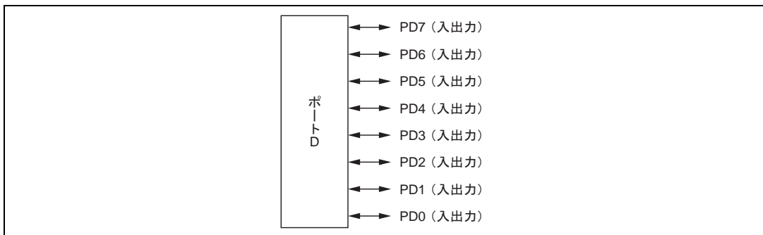
図 9.18 ポート D の端子機能 (モード 7)
