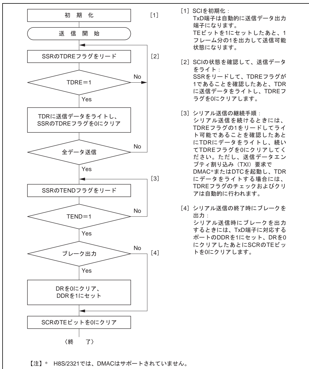
図 14.5 シリアル送信のフローチャートの例
