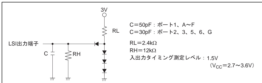
図 22.1 出力負荷回路
