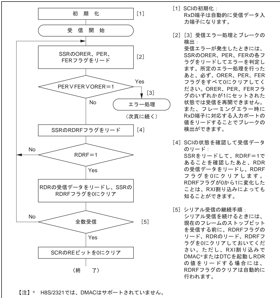
図 14.7 (1) シリアル受信フローチャートの例
