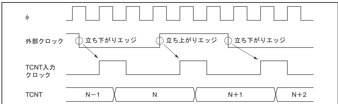
図 10.35 外部クロック動作時のカウンタタイミング
