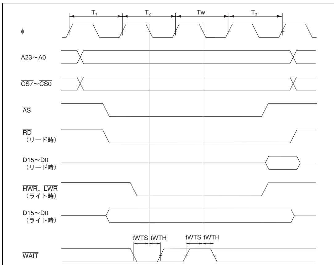
図 22.8 基本バスタイミング / 3 ステートアクセス 1 ウェイト
