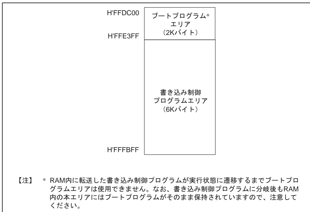
図 19.69 ブートモード時の RAM エリア
