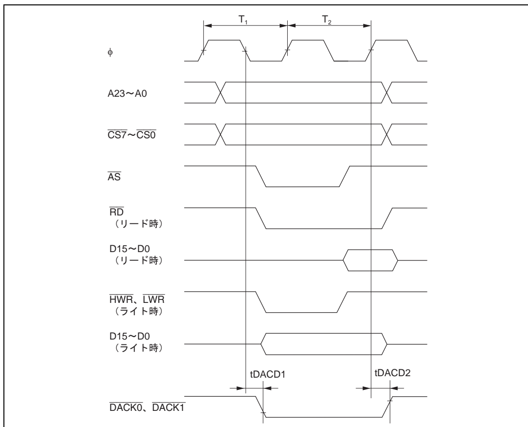
図 22.16 DMAC シングルアドレス転送タイミング / 2 ステートアクセス
