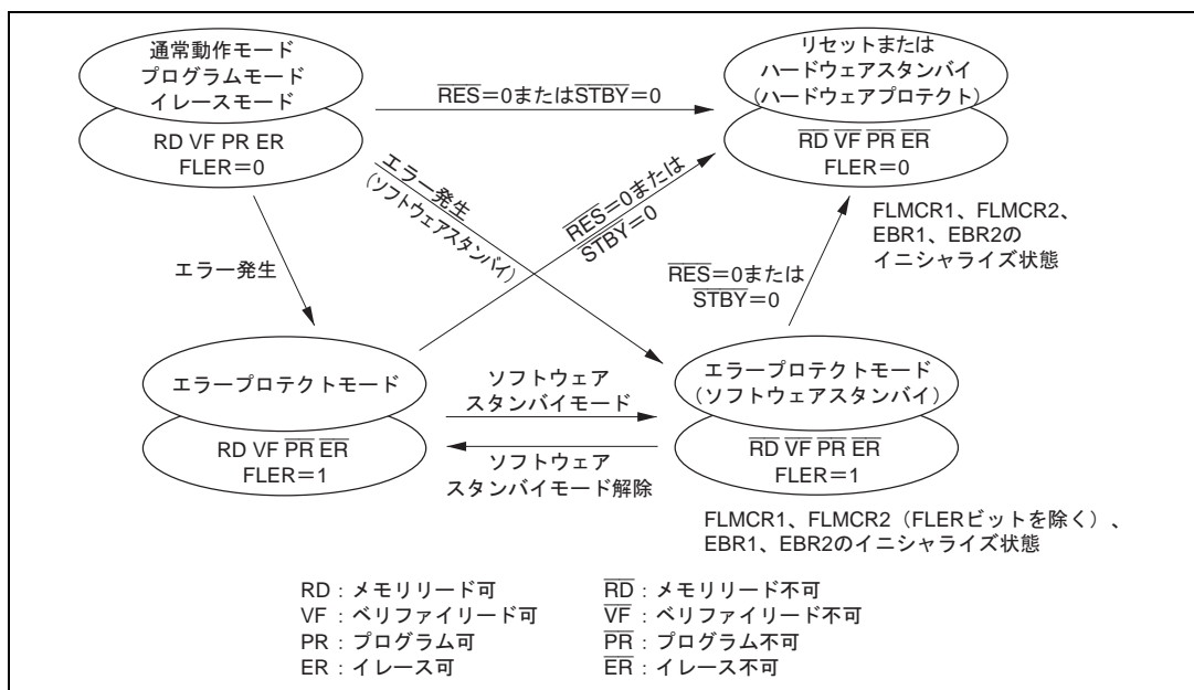
図 19.73 フラッシュメモリの状態遷移図
