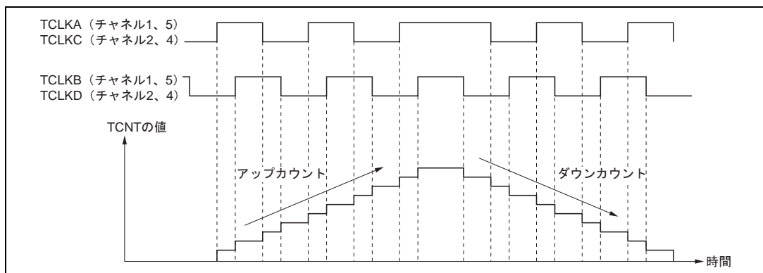
図 10.29 位相計数モード1の動作例
