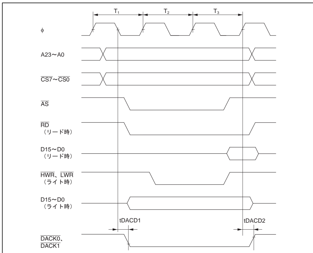
図 22.17 DMAC シングルアドレス転送タイミング / 3 ステートアクセス
