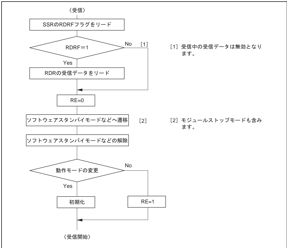
図 14.26 受信時のモード遷移フローチャートの例
