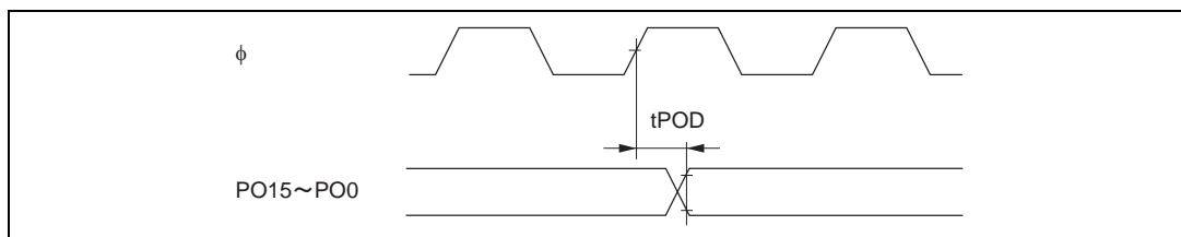
図 22.21 PPG 出力タイミング
