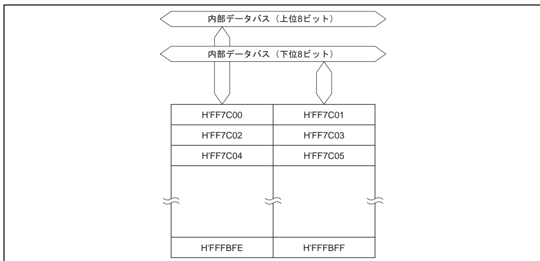
図 18.1 RAM のブロック図 (32K バイト)
