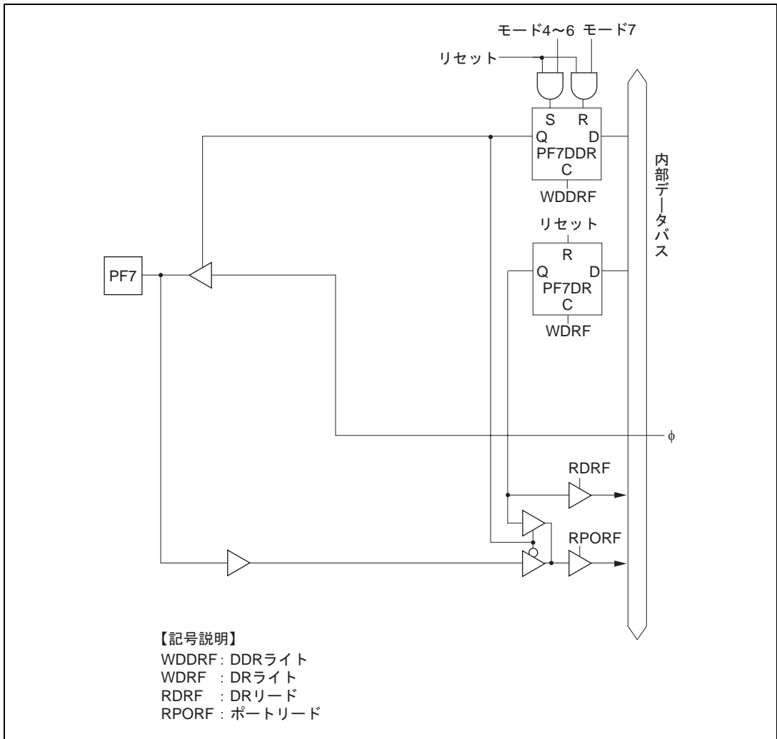
図 C.12 (h) ポート F ブロック図 (PF7 端子)
