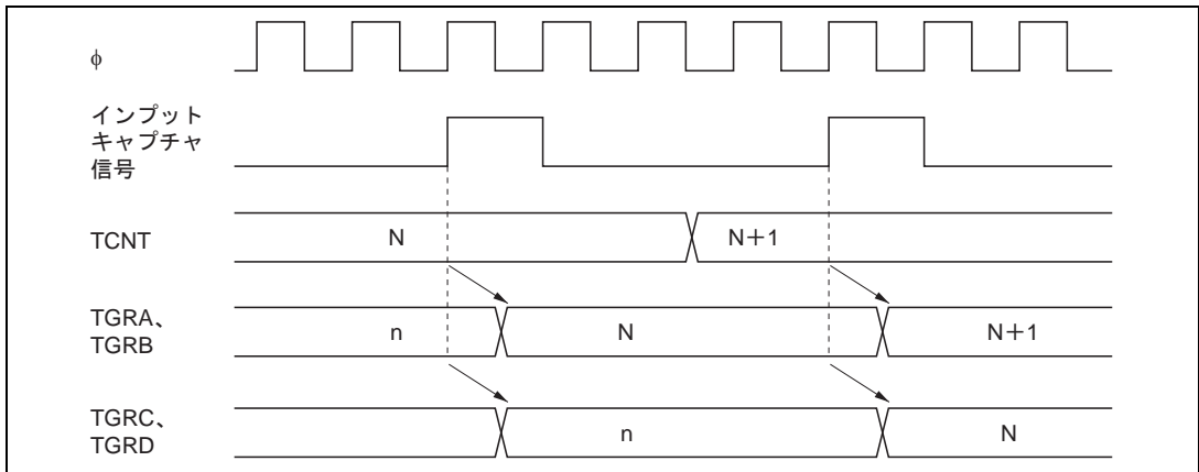
図 10.41 バッファ動作タイミング (インプットキャプチャ)
