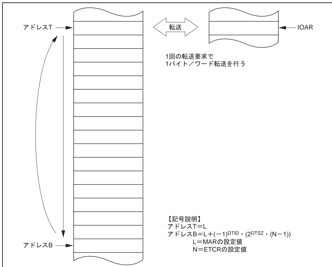
図 7.7 リピートモードの動作図
