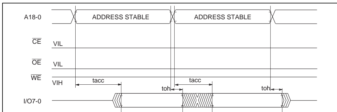
図 19.80 \overline{CE} 、 \overline{OE} イネーブル状態リード時のタイミング波形
