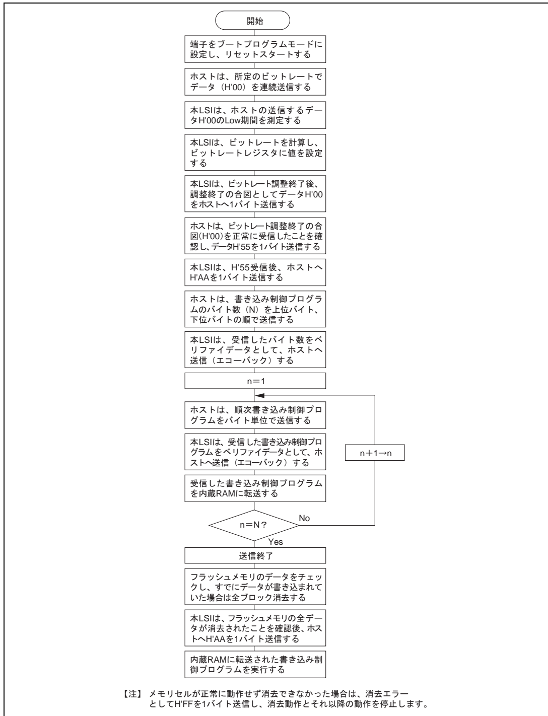
図 19.37 ブートモード実行手順
