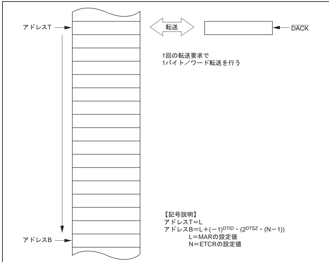
図 7.9 シングルアドレスモード（シーケンシャルモード指定時）の動作
