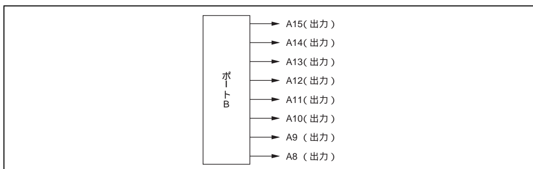
図 9.9 ポート B の端子機能 (モード 4、5)
