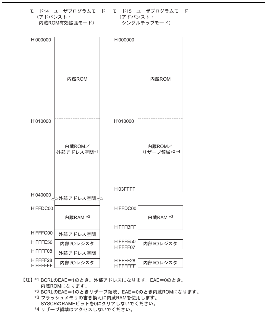
図 3.2 H8S/2328 の各動作モードのアドレスマップ (3) [ F-ZTAT 版のみ ]
