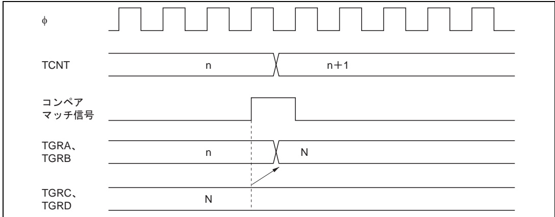
図 10.40 バッファ動作タイミング (コンペアマッチ)
