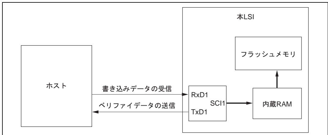
図 19.66 ブートモード時のシステム構成図
