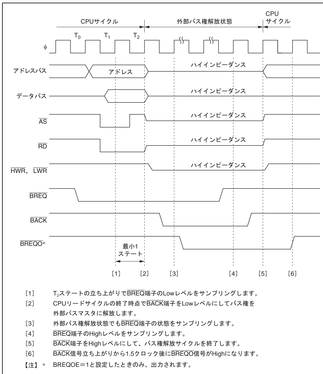
図 6.37 バス権解放状態遷移タイミング
