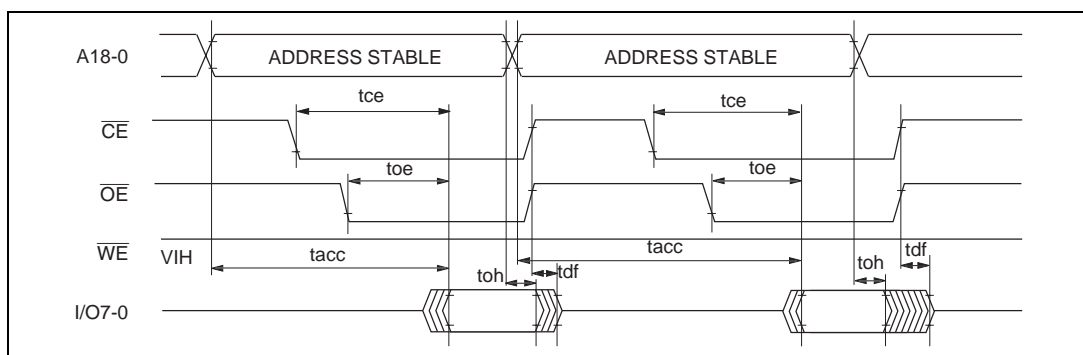
図 19.81 \overline{CE} 、 \overline{OE} クロック方式リード時のタイミング波形
