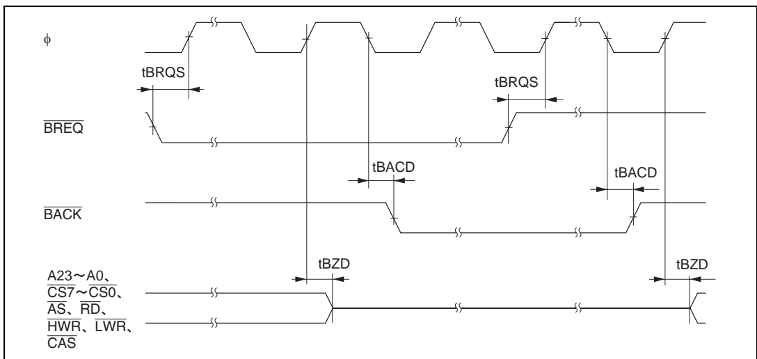
図 22.14 外部バス権解放タイミング
