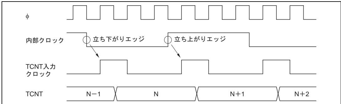
図 10.34 内部クロック動作時のカウンタタイミング
