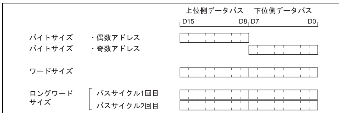
図 6.5 アクセスサイズとデータアライメント制御 (16 ビットアクセス空間)
