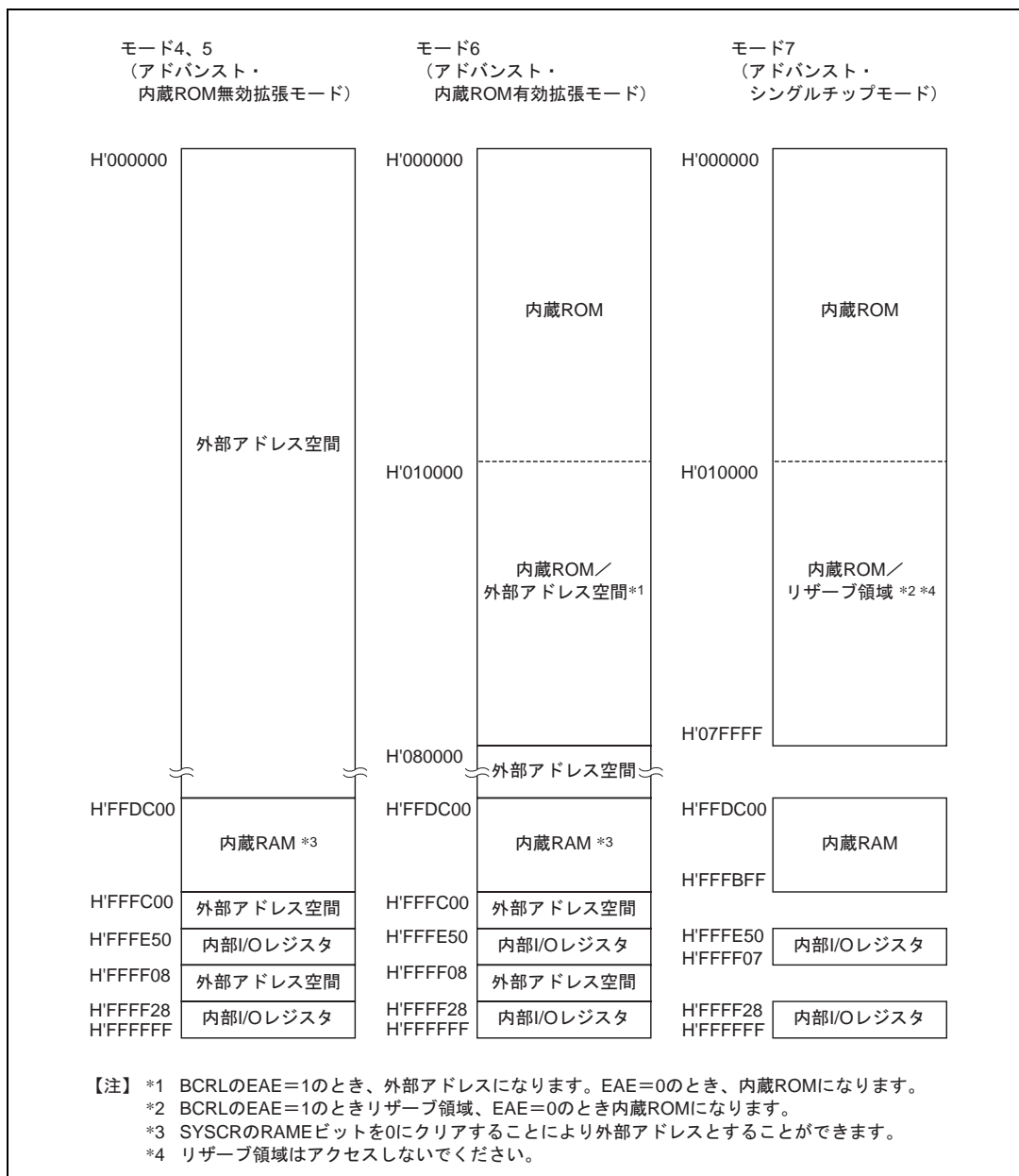
図 3.4 H8S/2326 F-ZTAT の各動作モードのアドレスマップ (1)
