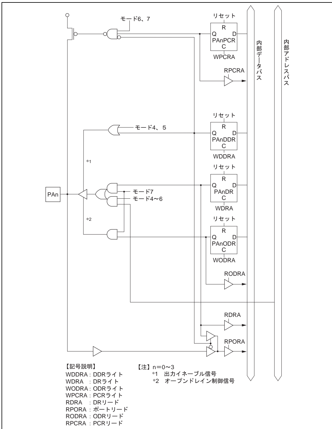
図 C.7 (a) ポート A ブロック図 (PA0 ~ PA3 端子)
