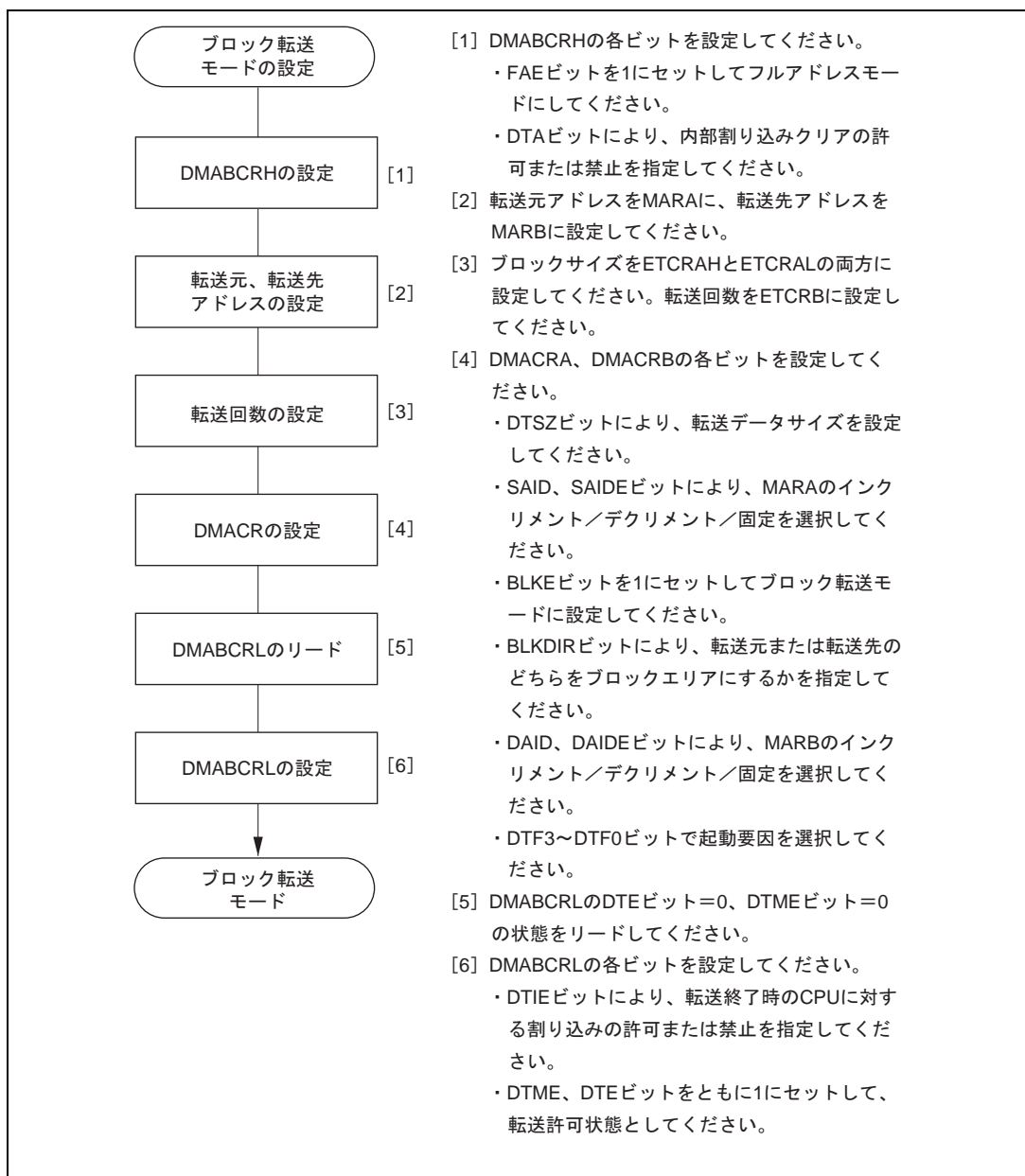
図 7.16 ブロック転送モードの設定手順例
