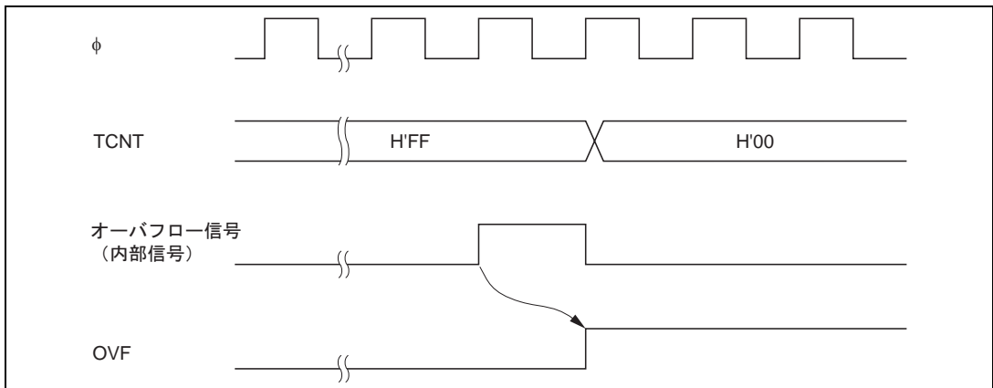
図 13.6 OVF のセットタイミング
