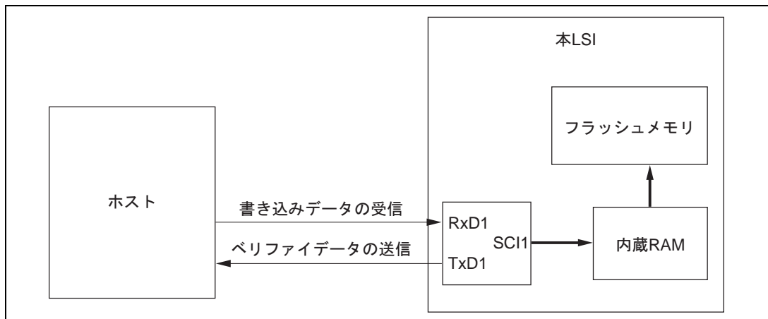
図 19.9 ブートモード時のシステム構成図
