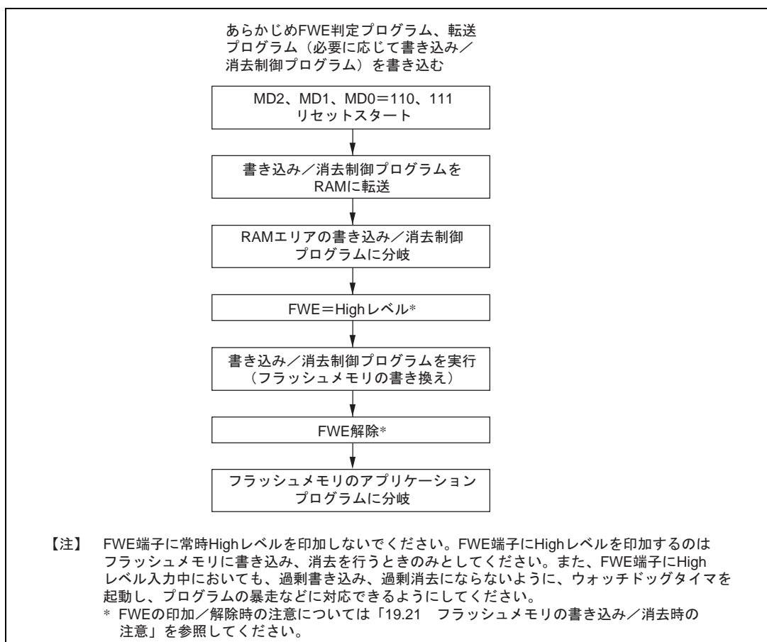
図 19.40 ユーザプログラムモードの実行手順例
