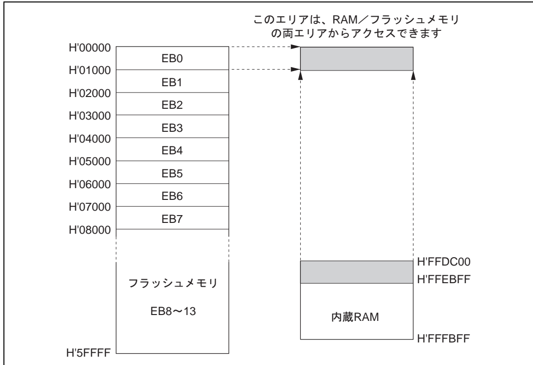
図 19.18 RAM のオーバーラップ動作例
