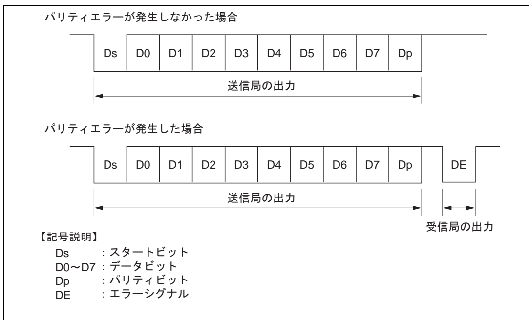
図 15.3 通常のスマートカードインターフェースのデータフォーマット
