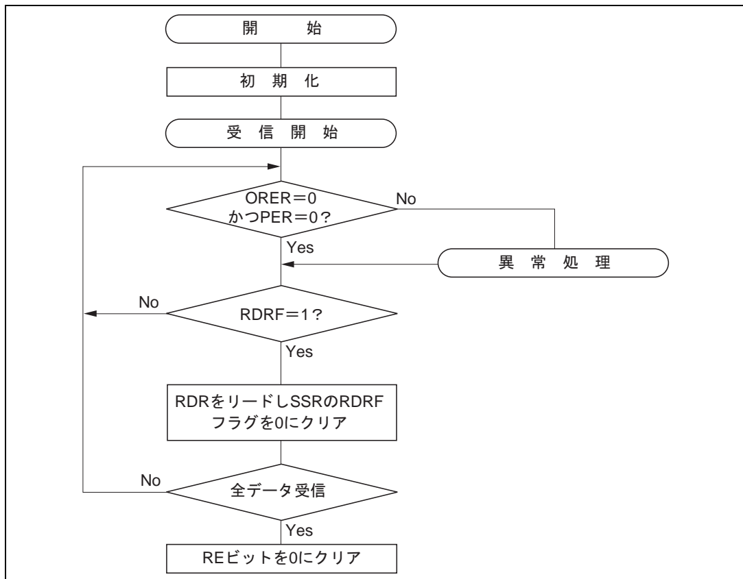
図 15.7 受信処理フローの例
