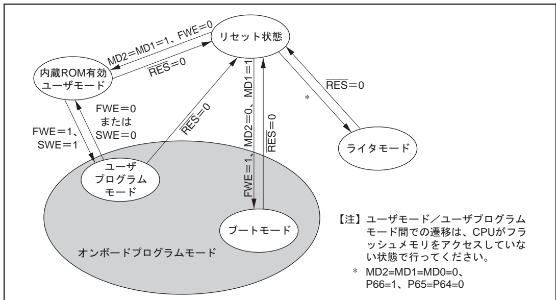
図 19.30 フラッシュメモリに関する状態遷移
