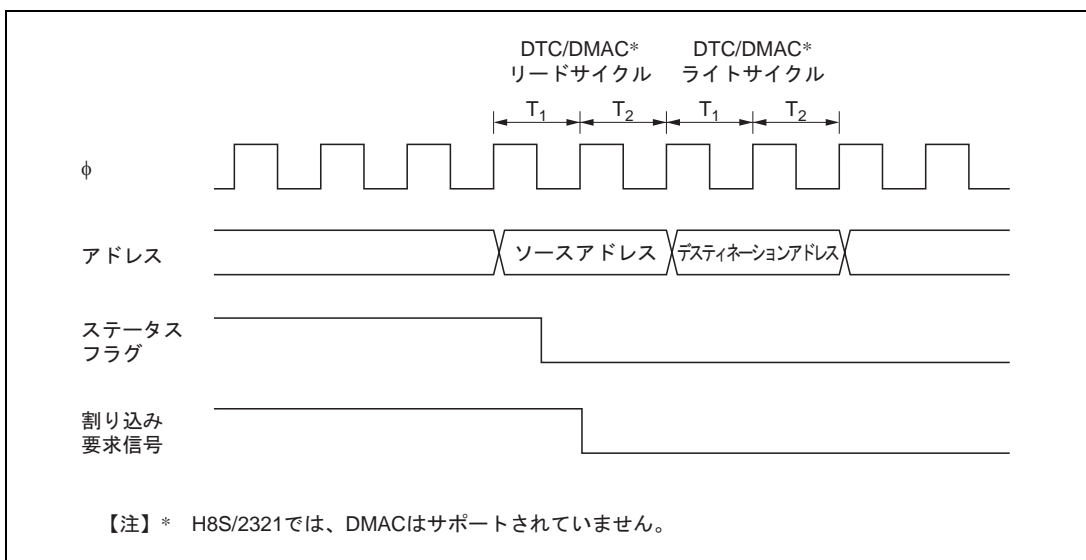
図 10.47 DTC/DMAC*の起動によるステータスフラグのクリアタイミング
