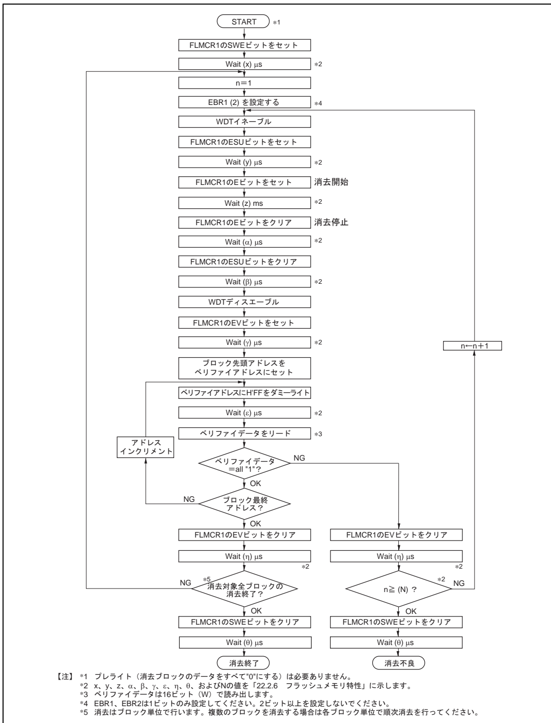
図 19.42 イレース/イレースペリファイフロー
