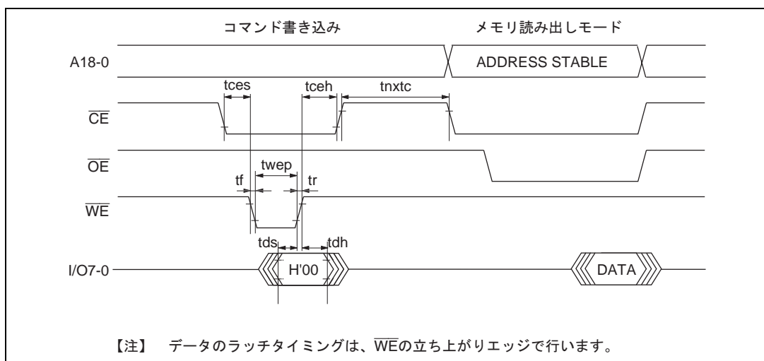
図 19.21 コマンド書き込み後メモリ読み出しタイミング波形
