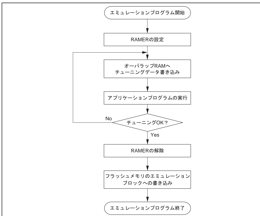
図 19.17 RAM によるエミュレーションフロー
