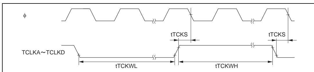
図 22.23 TPU クロック入力タイミング
