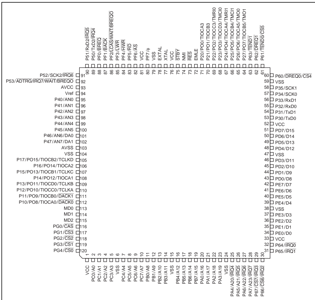
図 1.7 HD64F2329B ピン配置図 (TFP-120 : 上面図)
