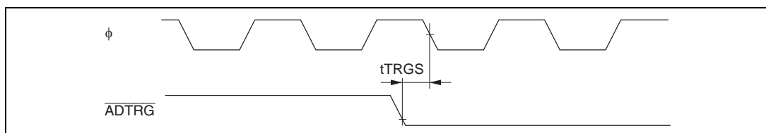
図 22.30 A/D 変換器外部トリガ入力タイミング
