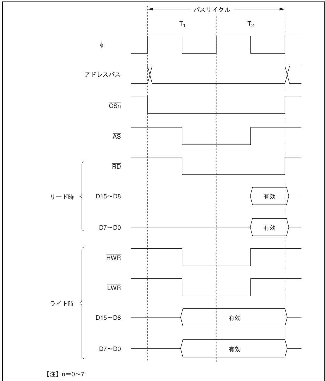
図 6.10 16 ビット 2 ステートアクセス空間のバスタイミング (3) (ワードアクセス)
