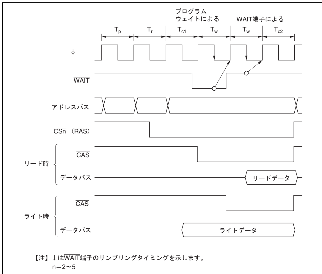
図 6.17 ウェイトステート挿入タイミング例
