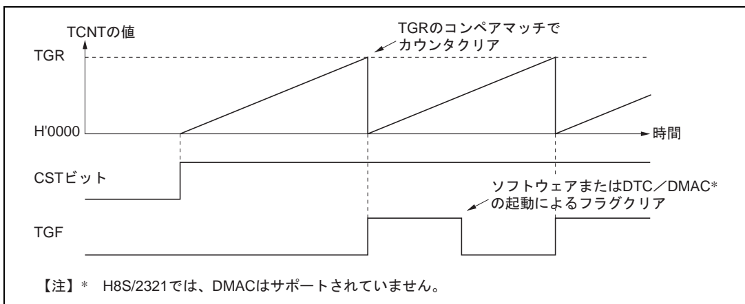
図 10.8 周期カウンタの動作
