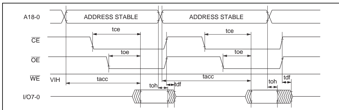
図 19.51 CE、OE クロック方式リード時のタイミング波形
