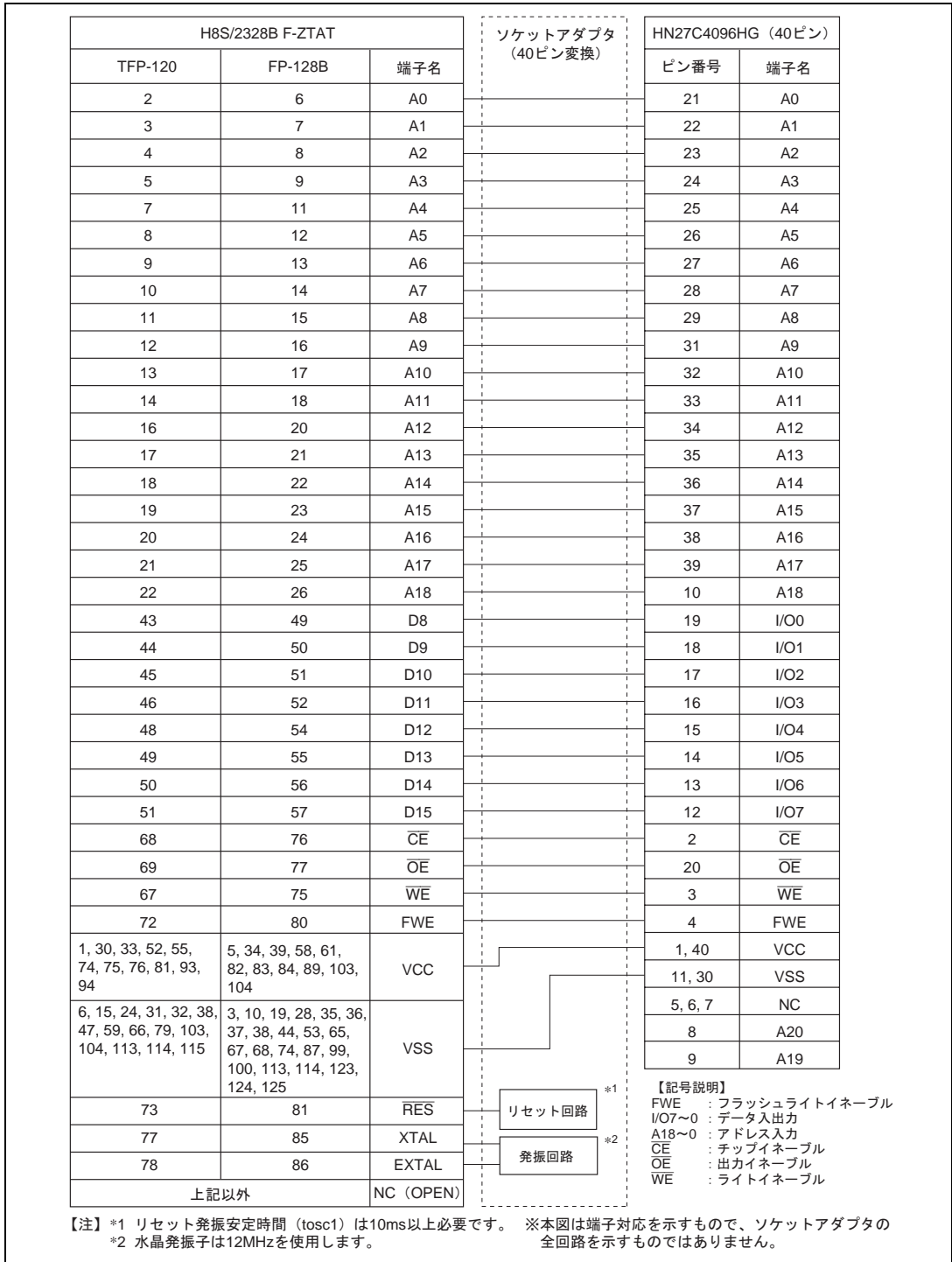
図 19.47 H8S/2328B F-ZTAT ソケットアダプタの端子対応図
