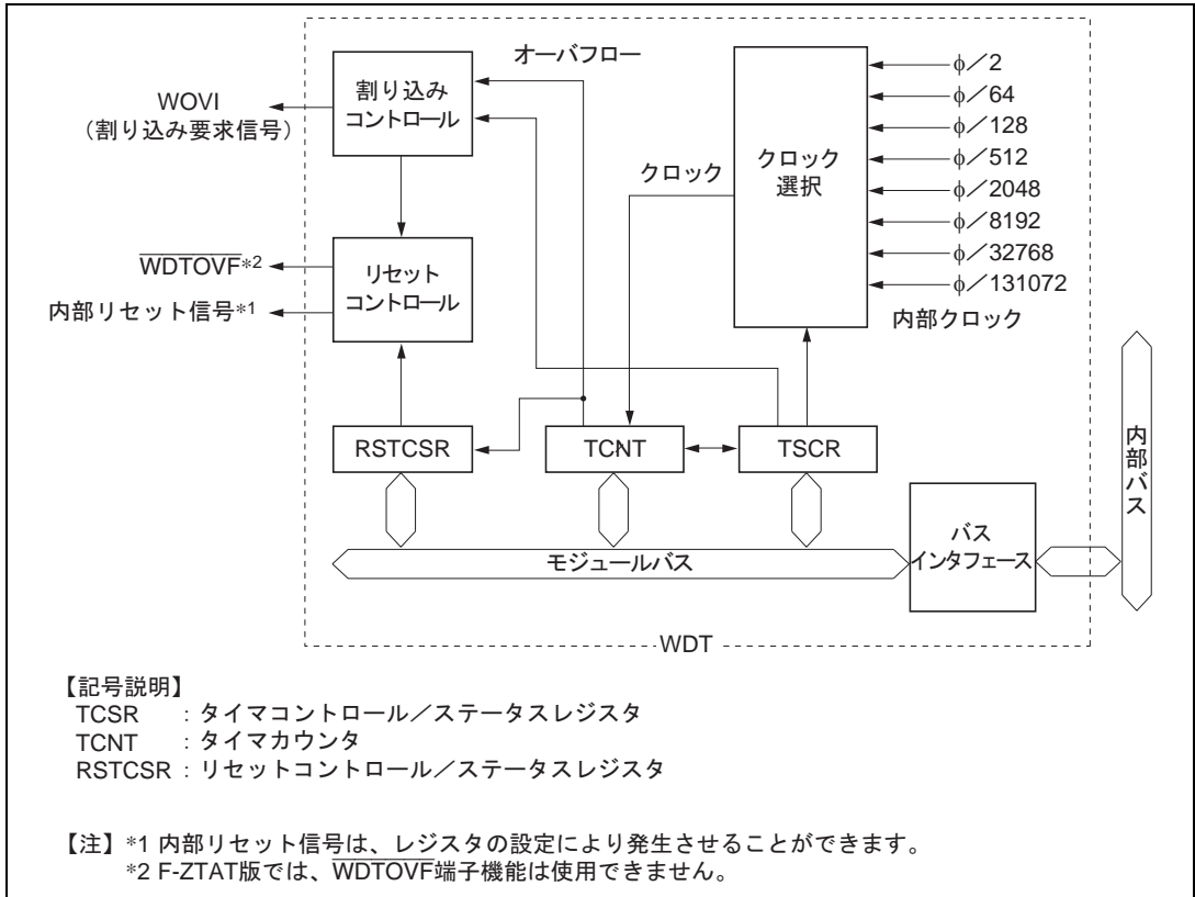
図 13.1 WDTのブロック図
