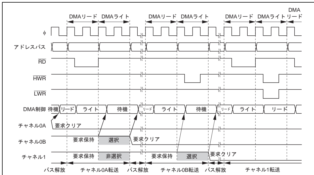
図 7.35 複数チャンネル転送例
