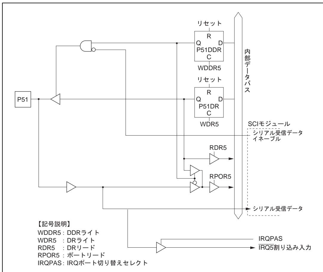
図 C.5 (b) ポート 5 ブロック図 (P51 端子)
