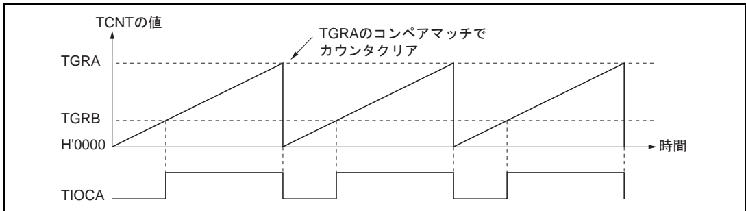
図 10.25 PWM モードの動作例 (1)
