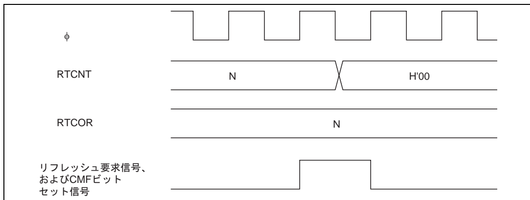
図 6.24 コンペアマッチのタイミング
