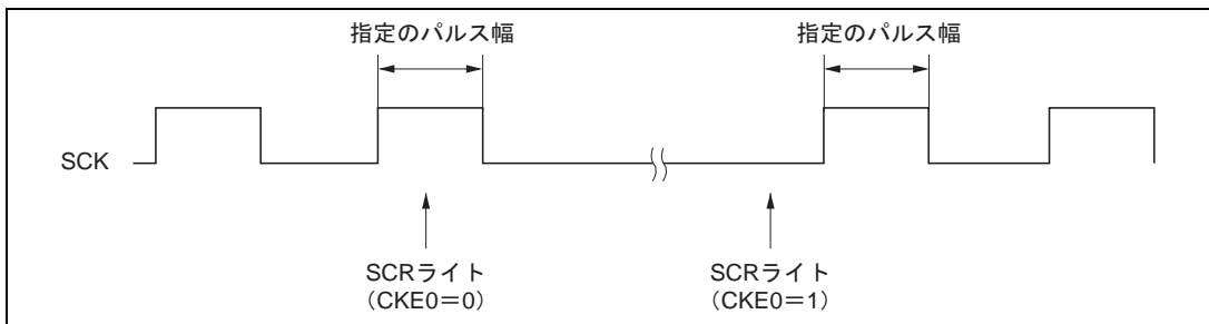
図 15.8 クロック出力固定タイミング
