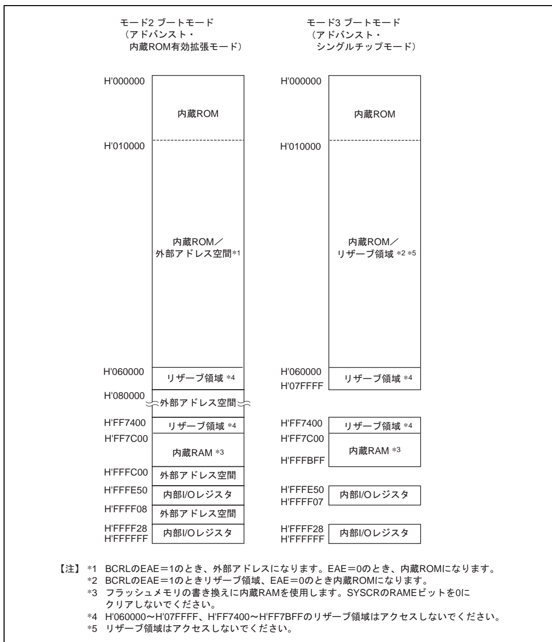
図 3.1 H8S/2329B の各動作モードのアドレスマップ (1)
