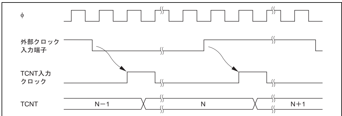
図 12.3 外部クロック動作時のカウントタイミング
