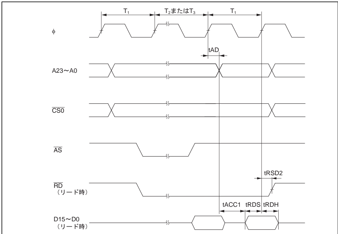
図 22.13 バーストROM アクセスタイミング / 1 ステートアクセス
