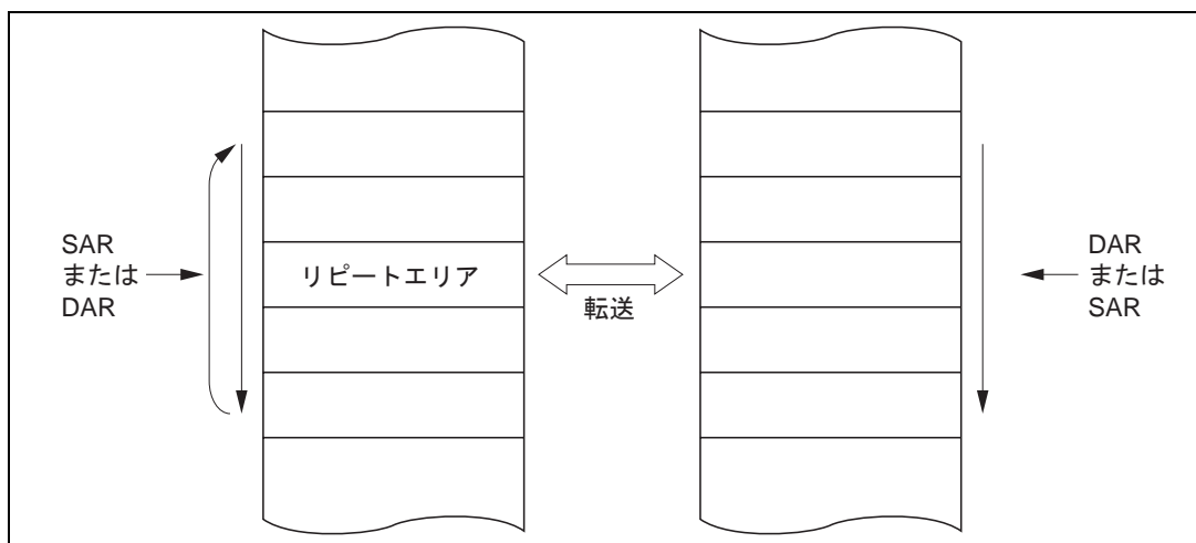
図 8.7 リピートモードのメモリマップ
