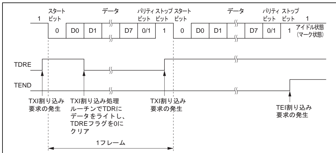
図 14.6 調歩同期式モードでの送信時の動作例 (8ビットデータ/パリティあり/1ストップビットの例)
