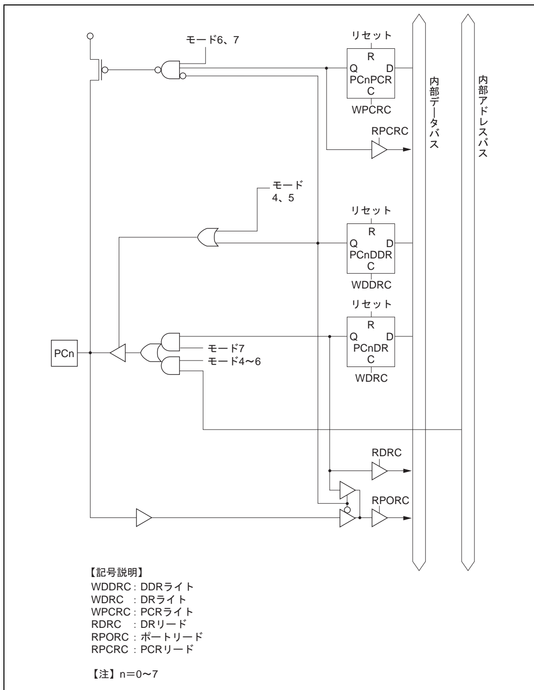
図 C.9 ポート C ブロック図 (PC0 ~ PC7 端子)
