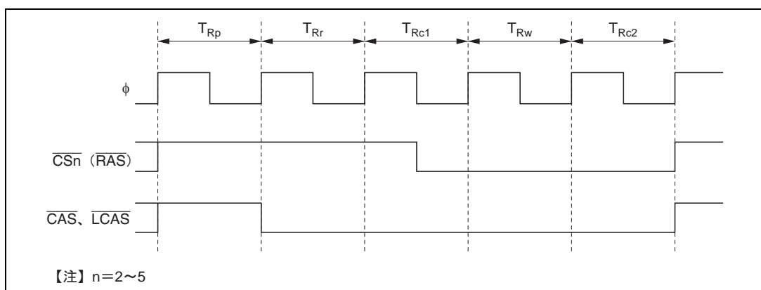
図 6.26 CBR リフレッシュタイミング (RCW=1、RLW1=0、RLW0=1 の場合)
