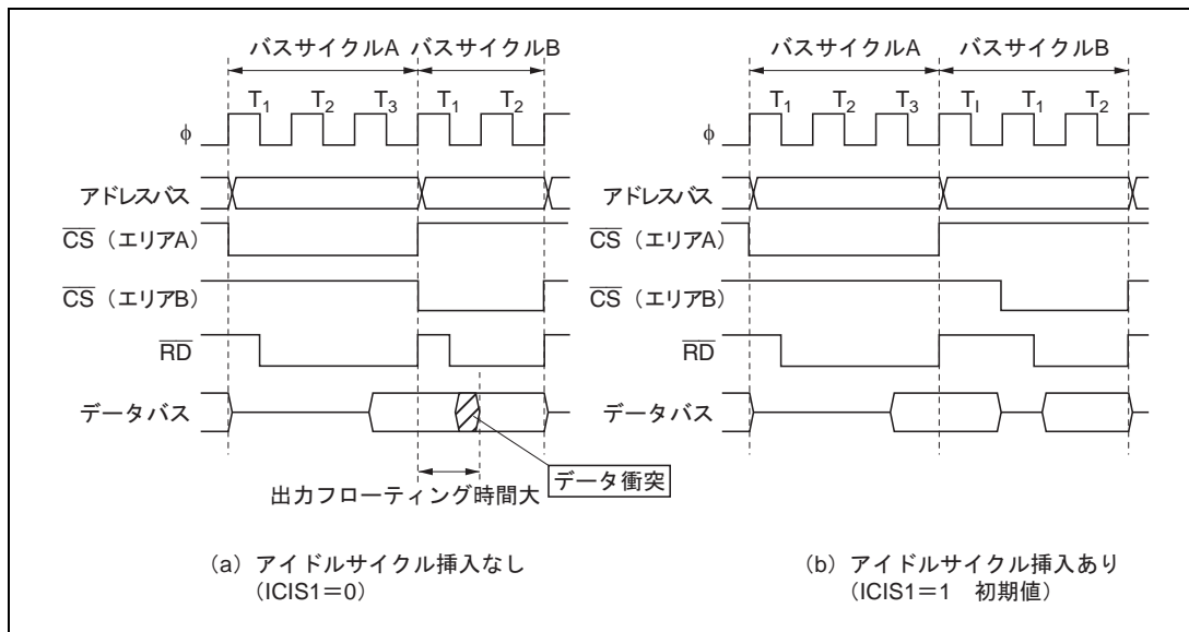
図 6.31 アイドルサイクル動作例 (1)
