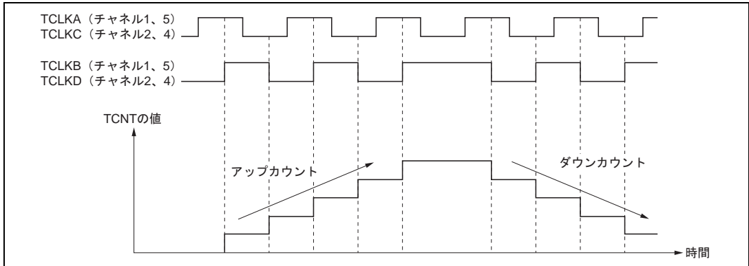
図 10.32 位相計数モード4の動作例
