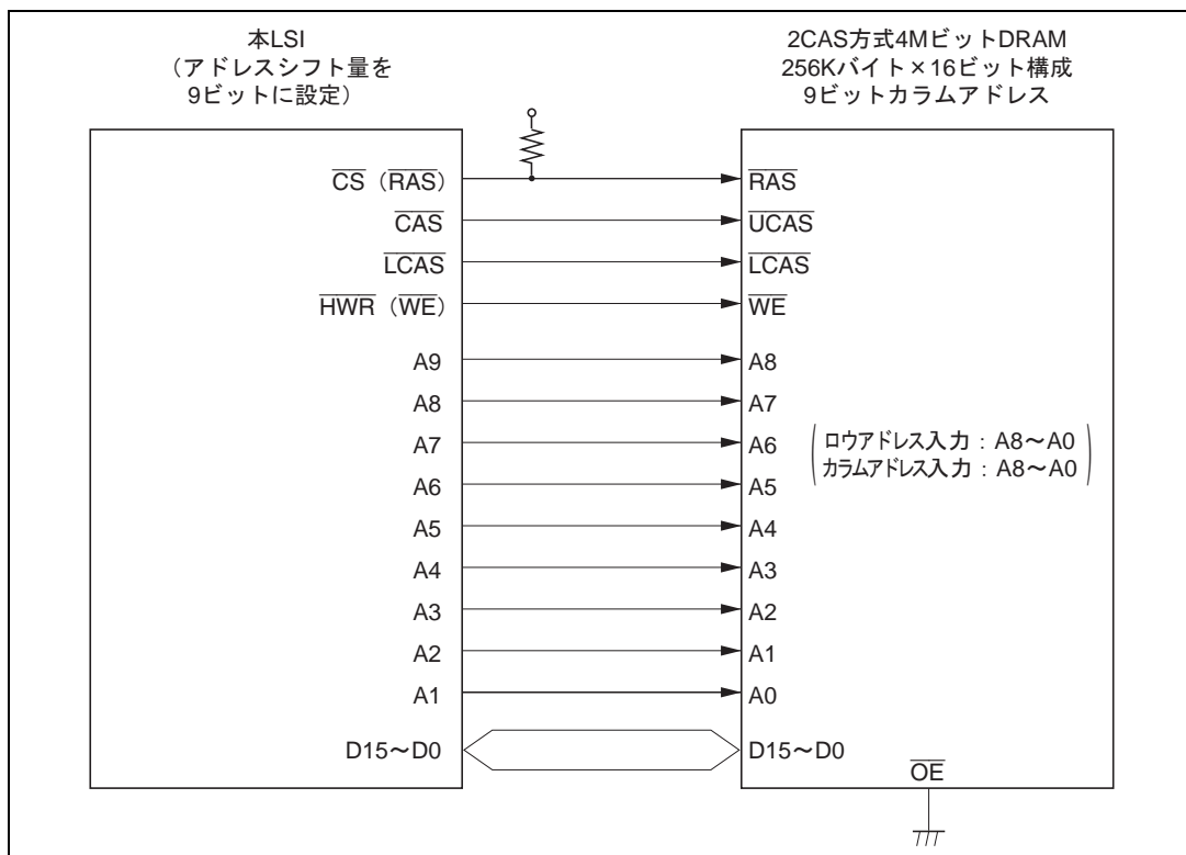
図 6.19 CAS2 本方式の接続例
