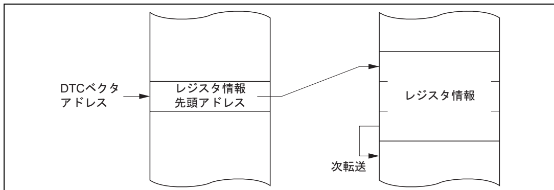
図 8.4 DTC ベクタアドレスとレジスタ情報との対応
