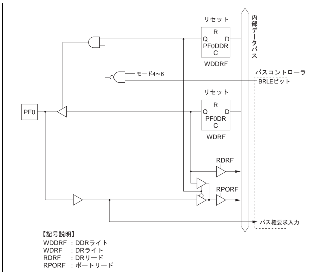
図 C.12 (a) ポート F ブロック図 (PF0 端子)
