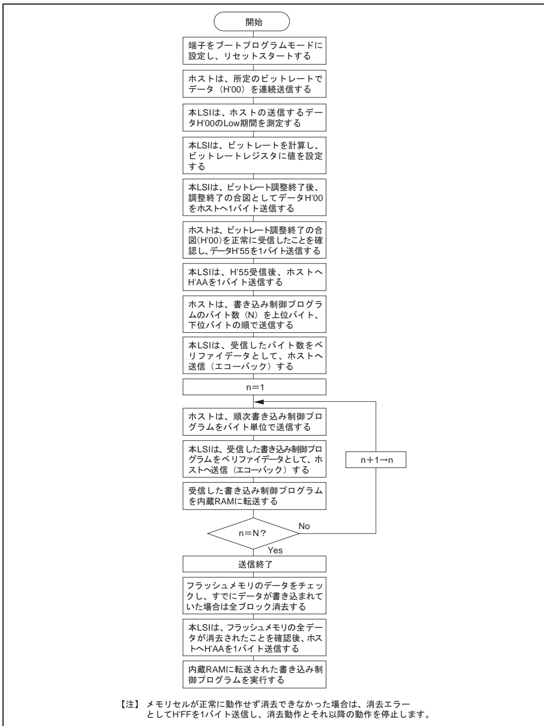
図 19.10 ブートモード実行手順
