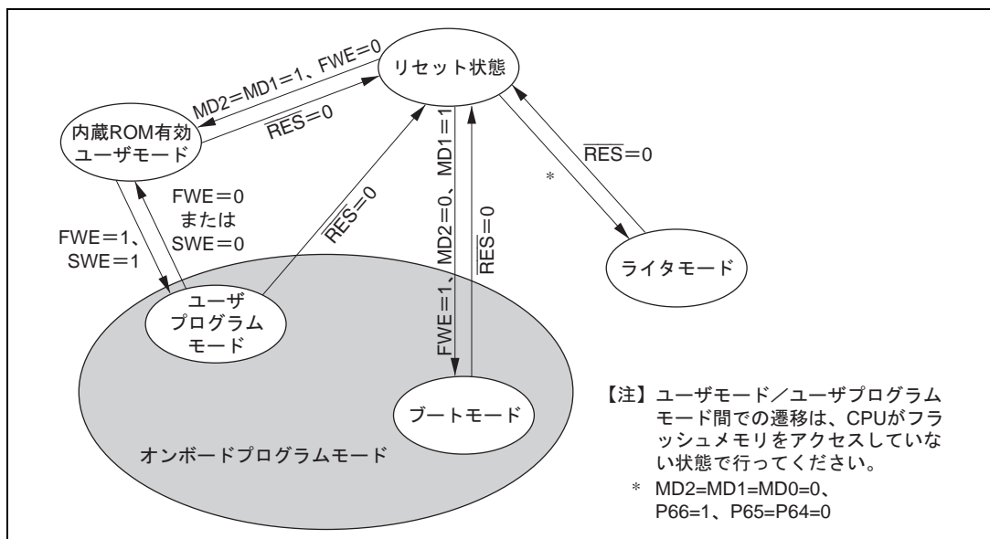
図 19.60 フラッシュメモリに関する状態遷移
