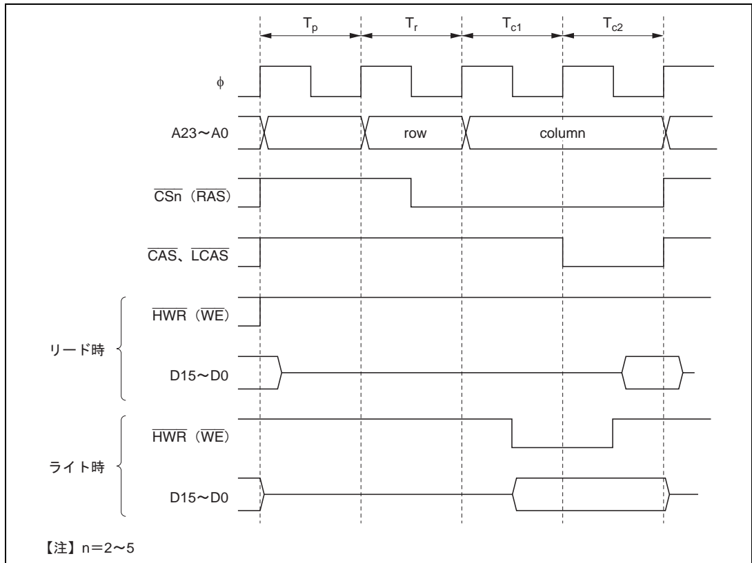
図 6.15 基本アクセスタイミング
