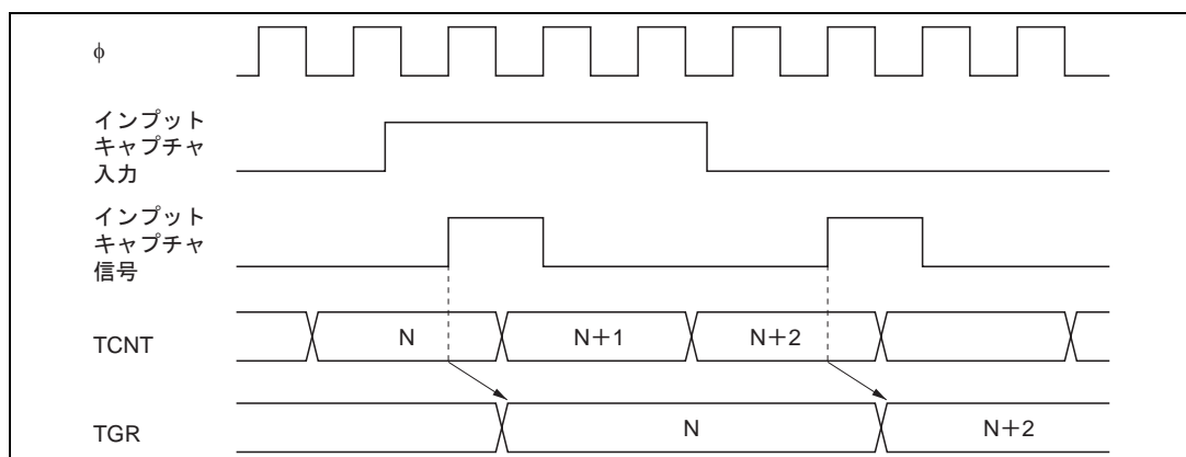
図 10.37 インพุットキャプチャ入力信号タイミング
