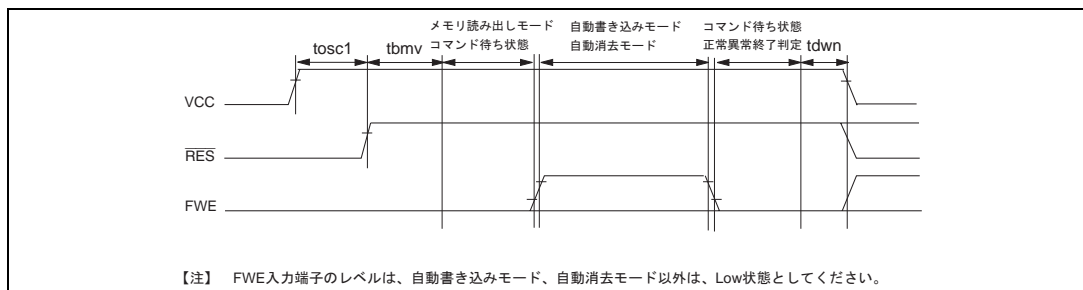
図 19.85 発振安定時間、ライタモードセットアップ、電源立ち下げシーケンス
