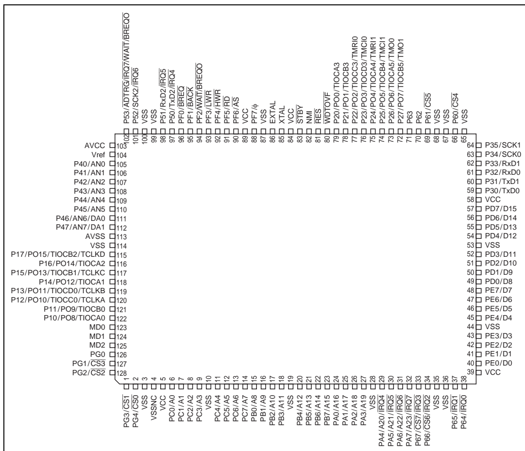
図 1.6 H8S/2321 ピン配置図 (FP-128B : 上面図)
