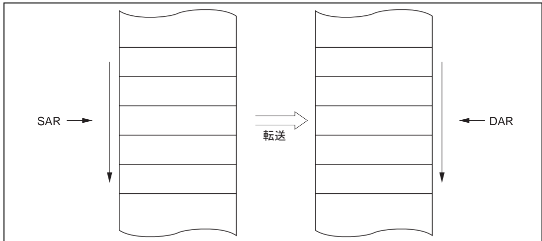
図 8.6 ノーマルモードのメモリマップ
