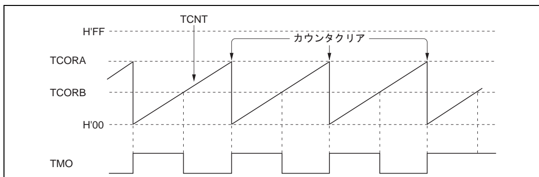
図 12.9 パルス出力例
