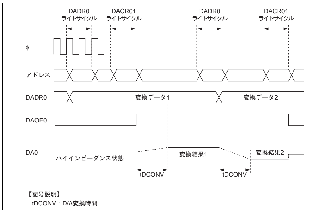
図 17.2 D/A 変換器の動作例
