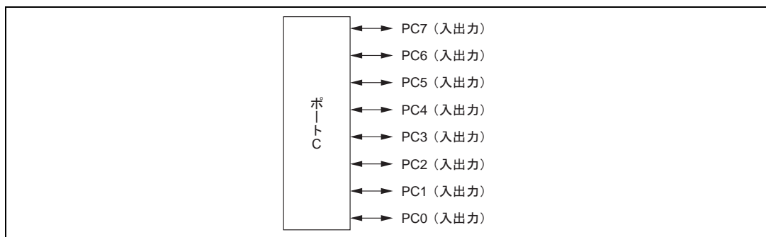
図 9.15 ポート C の端子機能 (モード 7)
