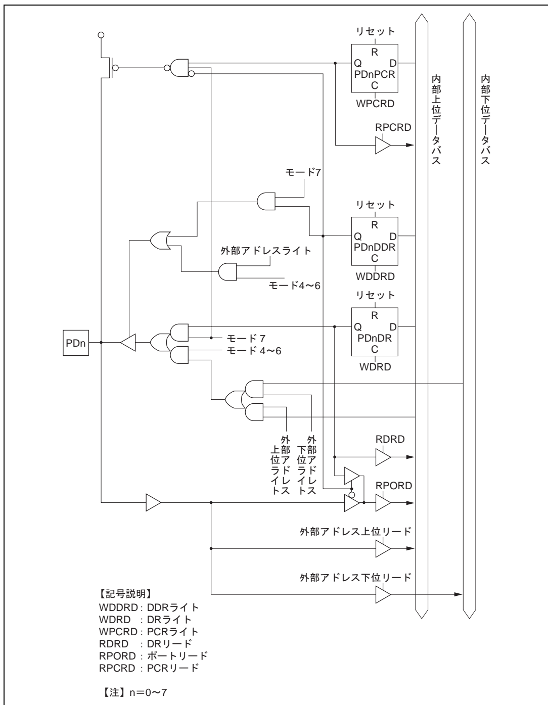
図 C.10 ポート D ブロック図 (PD0~PD7 端子)
