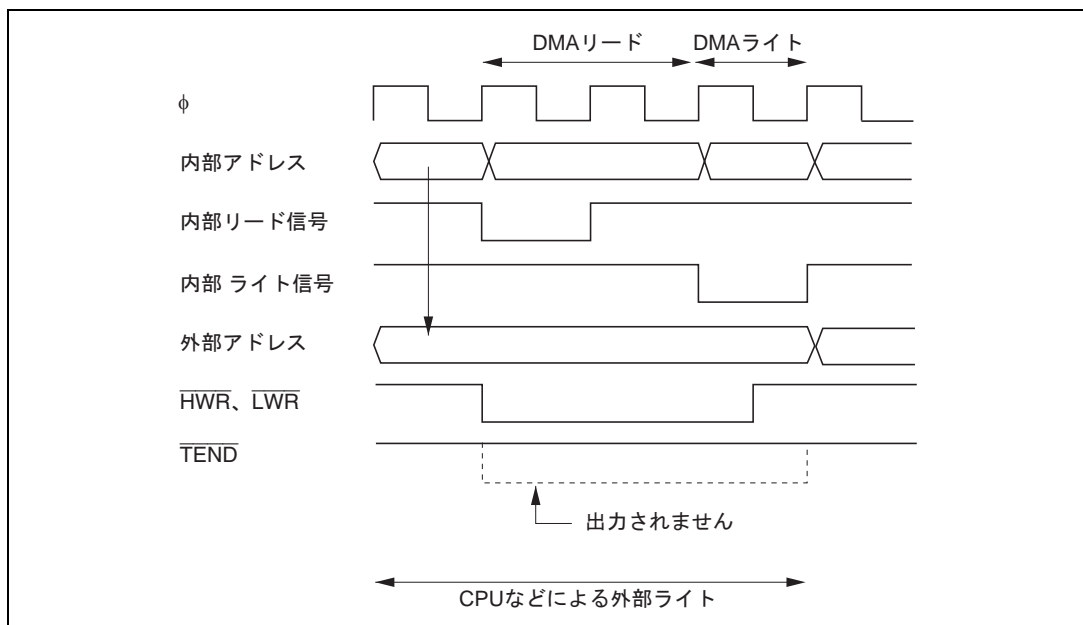
図 7.42 \overline{\text{TEND}} 端子に Low レベルが出力されない例
