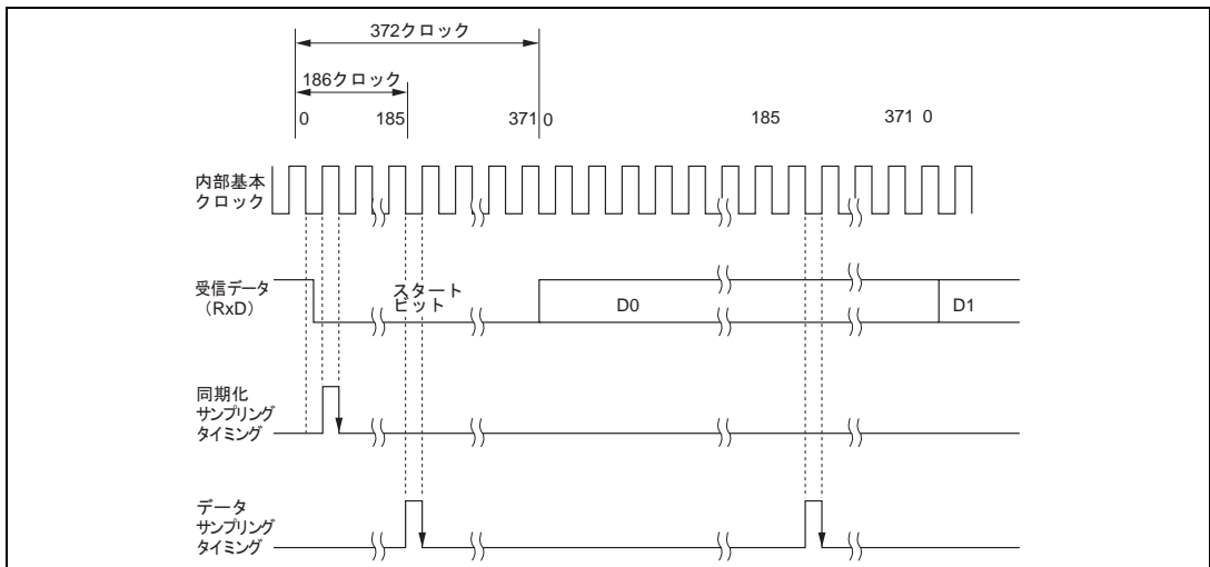
図 15.10 スマートカードインタフェースモード時の受信データサンプリングタイミング (372 倍のクロック使用時)
