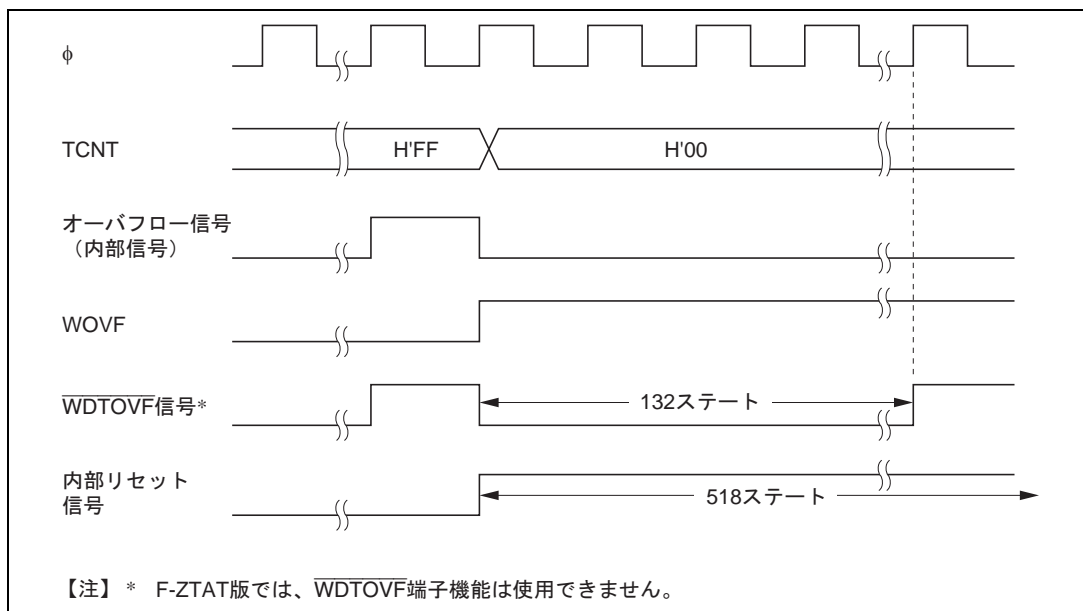
図 13.7 WOVF のセットタイミング
