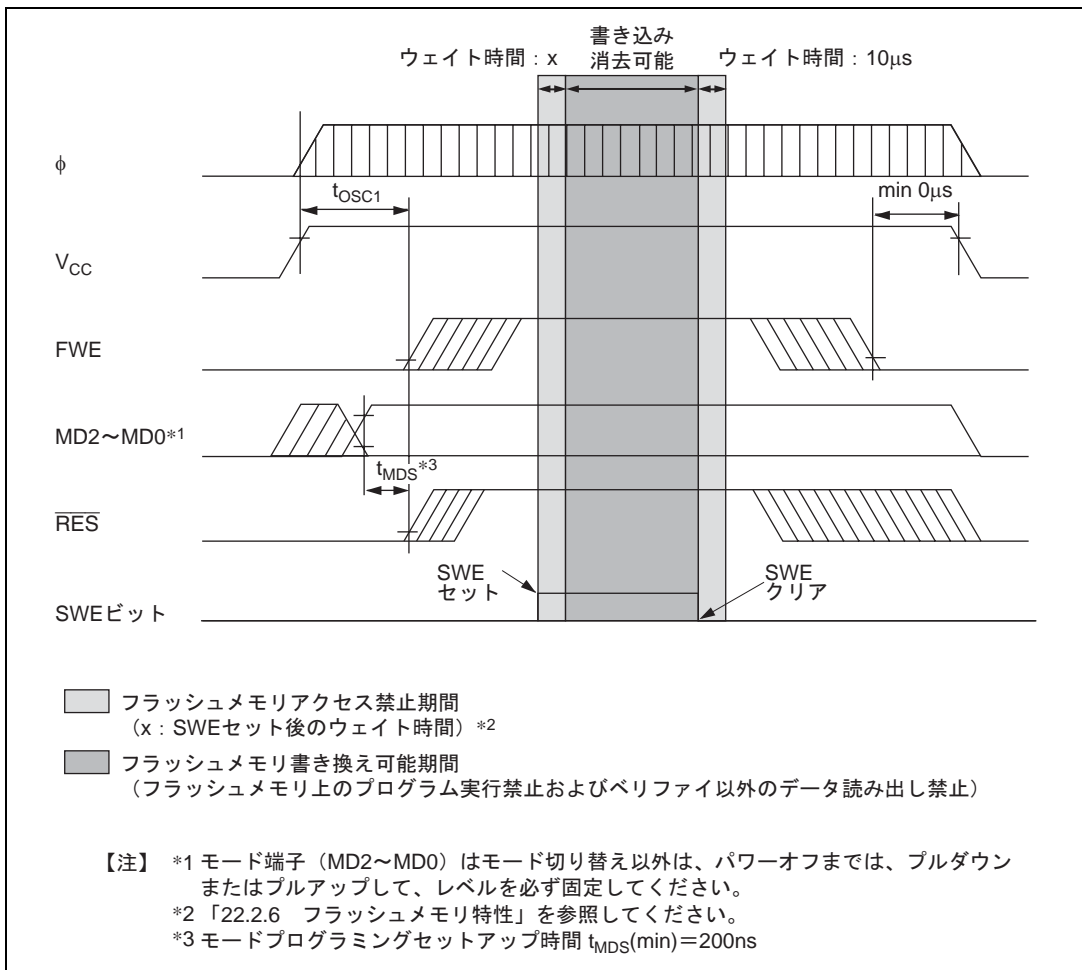
図 19.87 電源投入/切断タイミング (ユーザプログラムモード)
