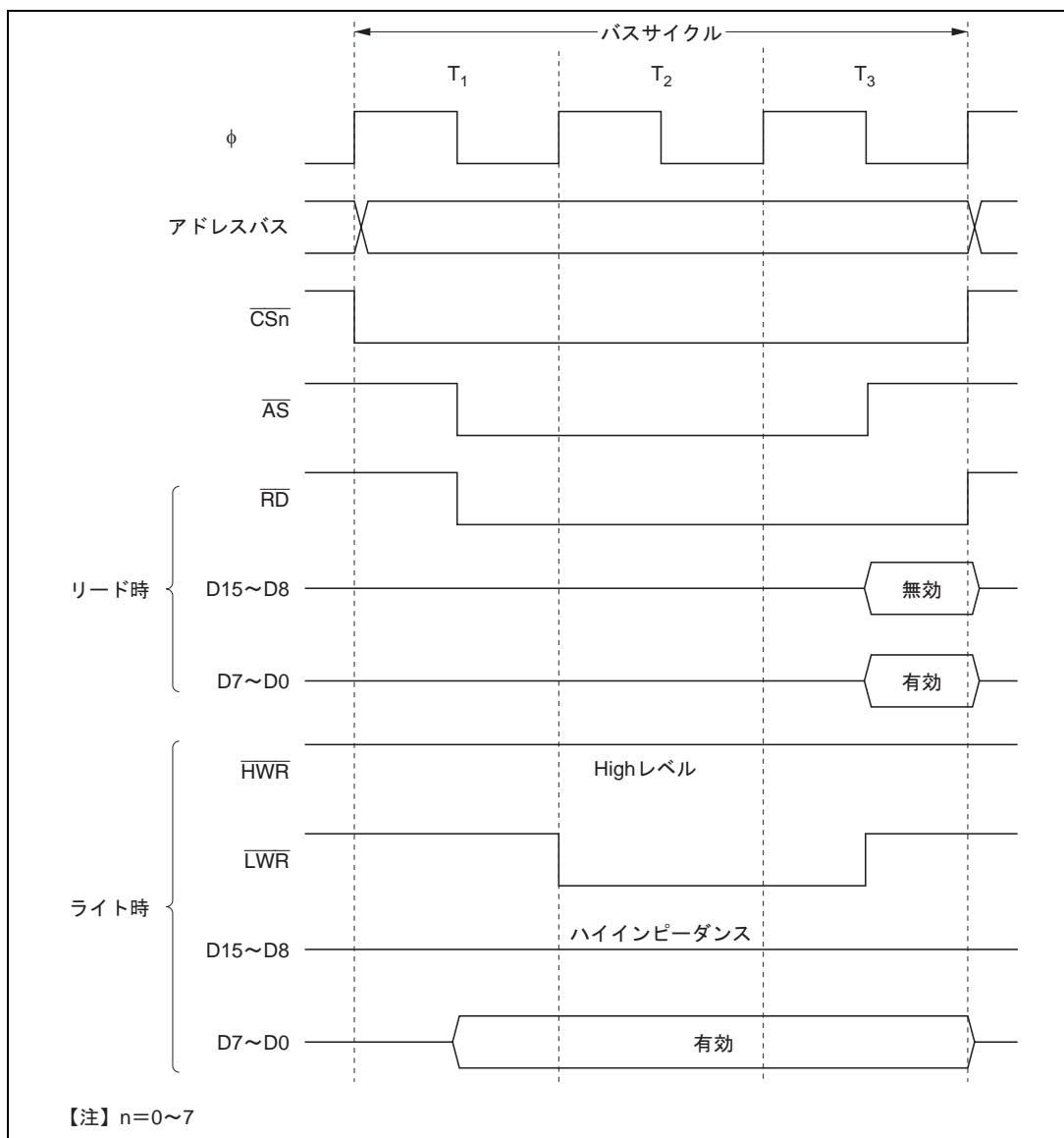
図 6.12 16 ビット 3 ステートアクセス空間のバスタイミング (2) (奇数アドレスバイトアクセス)
