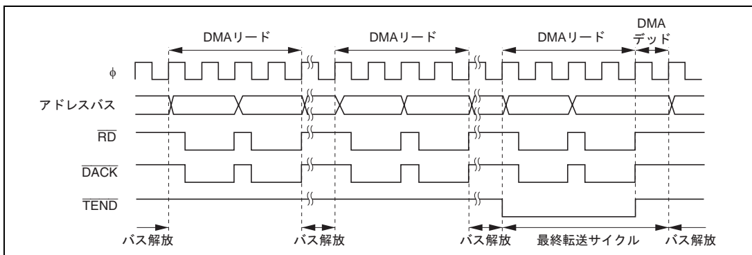
図 7.28 シングルアドレスモード (ワードリード) 転送例
