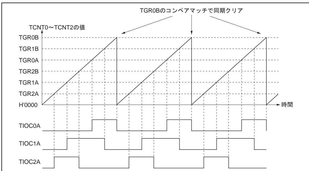
図 10.15 同期動作の動作例
