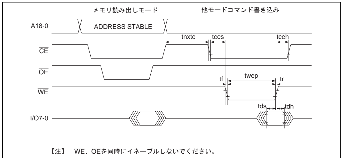
図 19.79 メモリ読み出しモードから他のモードへ遷移時のタイミング波形
