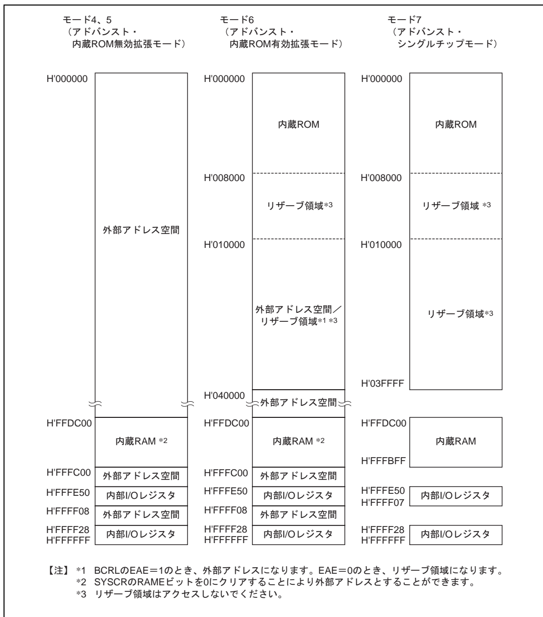
図 3.6 H8S/2323 の各動作モードのアドレスマップ
