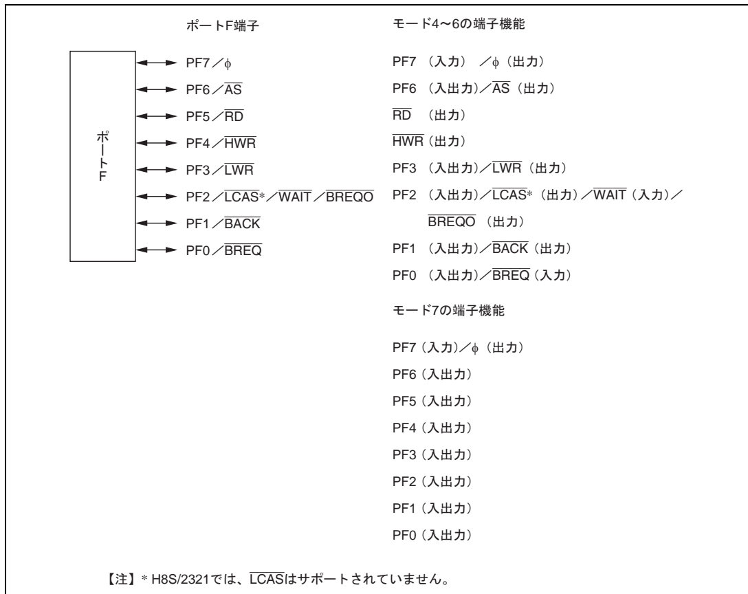
図 9.22 ポート F の端子機能
