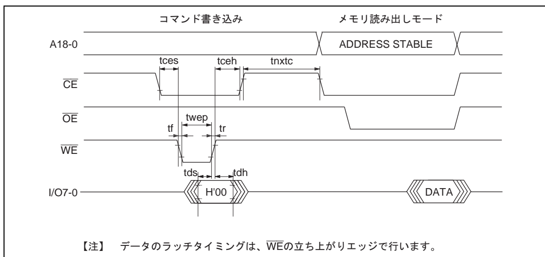
図 19.78 コマンド書き込み後メモリ読み出しタイミング波形
