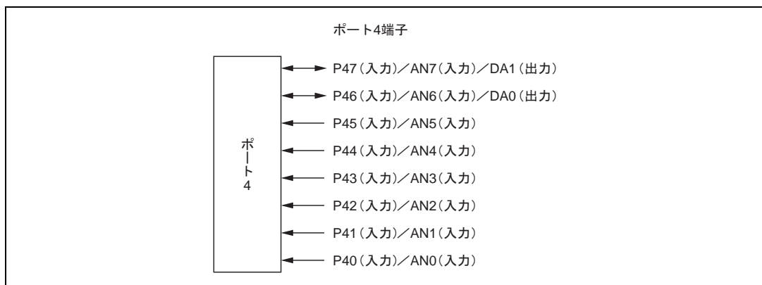
図 9.4 ポート 4 の端子機能
