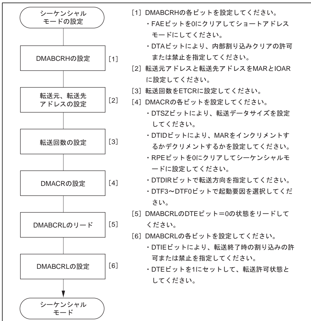
図 7.4 シーケンシャルモードの設定手順例
