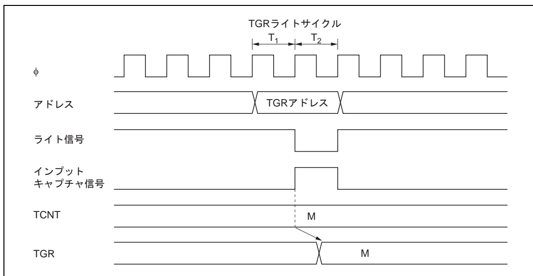
図 10.54 TGR のライトとインプットキャプチャの競合
