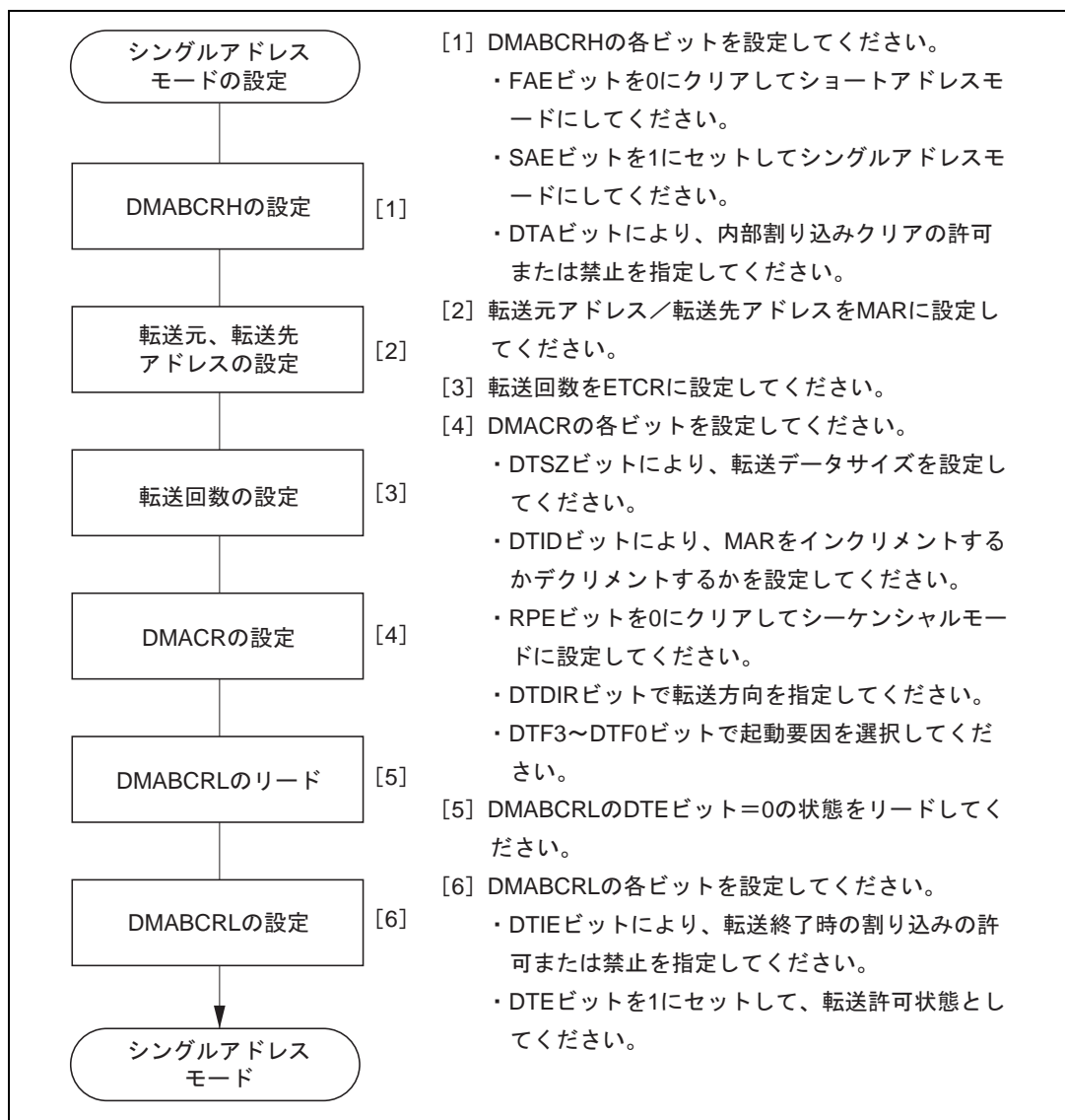
図 7.10 シングルアドレスモード（シーケンシャルモード指定）の設定手順例
