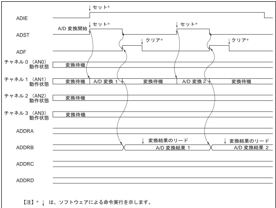
図 16.3 A/D 変換器の動作例（シングルモード、チャンネル 1 選択時）
