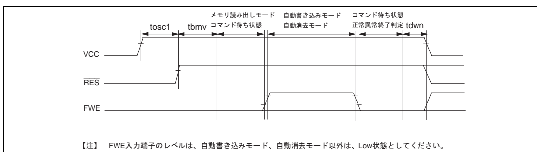
図 19.55 発振安定時間、ライタモードセットアップ、電源立ち下げシーケンス
