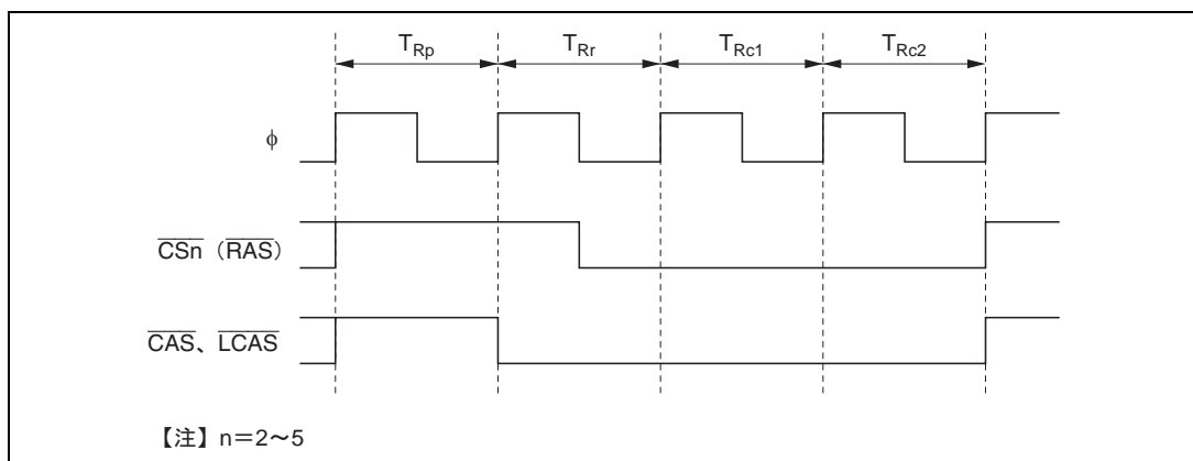
図 6.25 CBR リフレッシュタイミング
