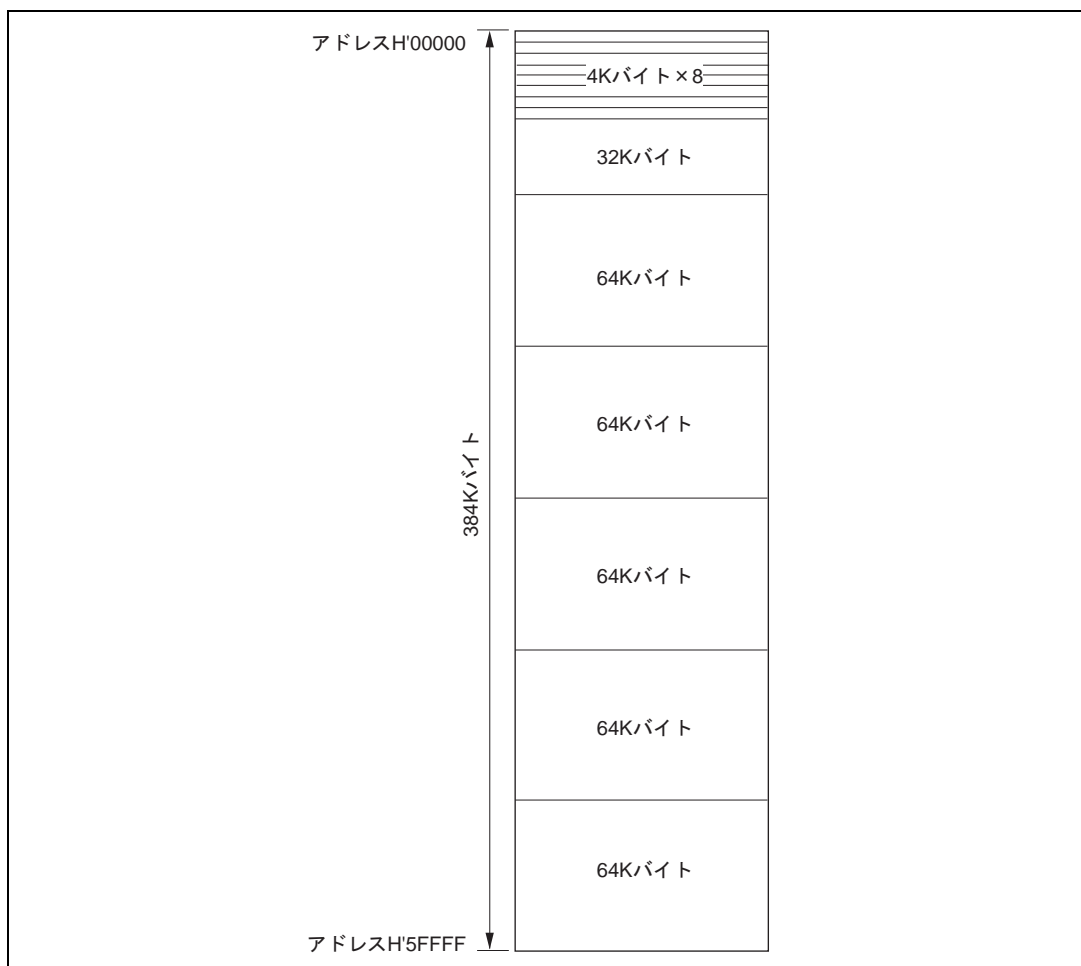
図 19.8 ブロック分割法
