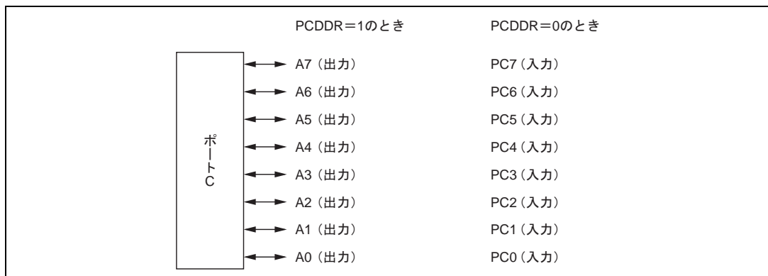
図 9.14 ポートCの端子機能（モード6）
