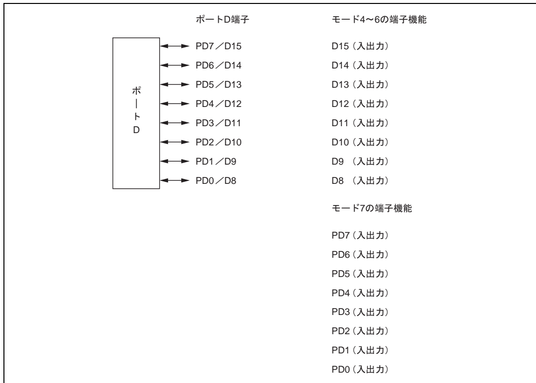
図 9.16 ポート D の端子機能
