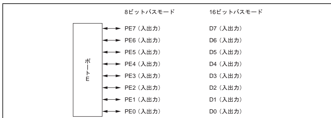
図 9.20 ポート E の端子機能 (モード 4~6)
