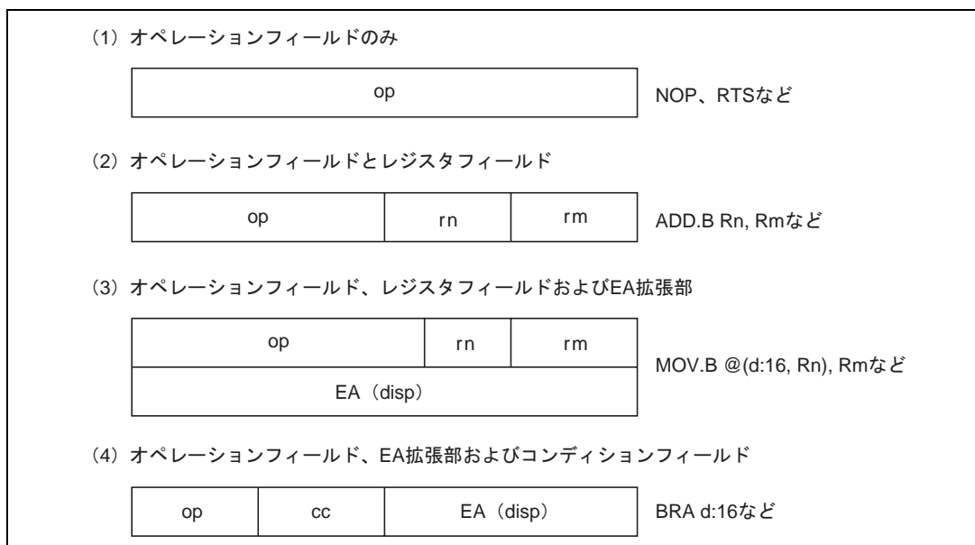
図 2.9 命令フォーマットの例
