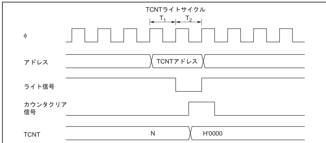
図 10.49 TCNTのライトとクリアの競合
