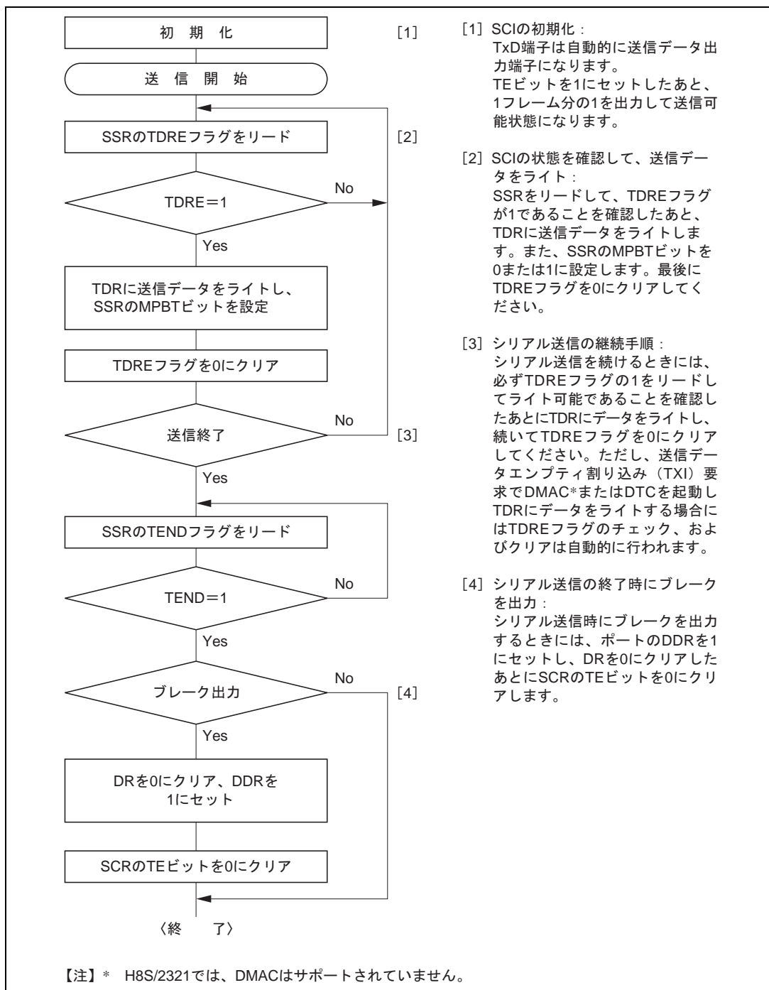
図 14.10 マルチプロセッサシリアル送信のフローチャートの例
