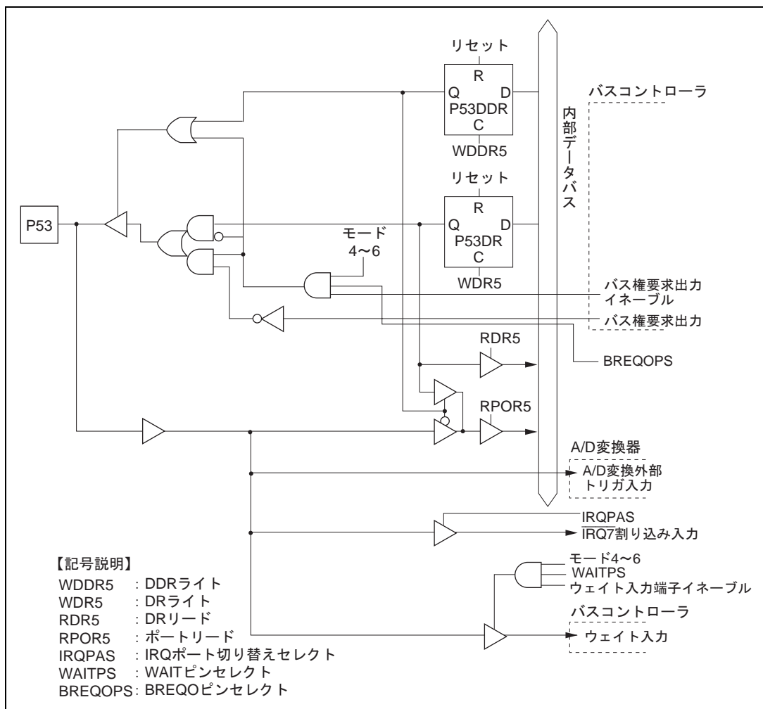
図 C.5 (d) ポート5ブロック図 (P53 端子)
