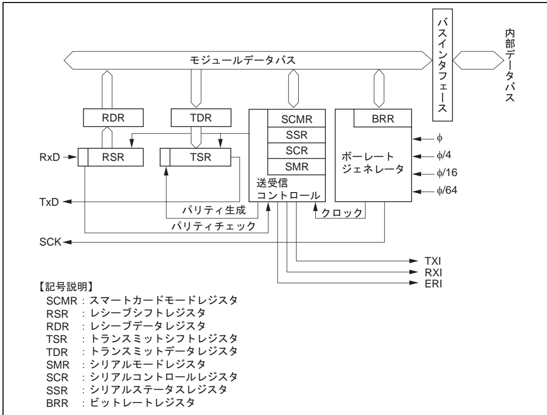
図 15.1 スマートカードインタフェースのブロック図
