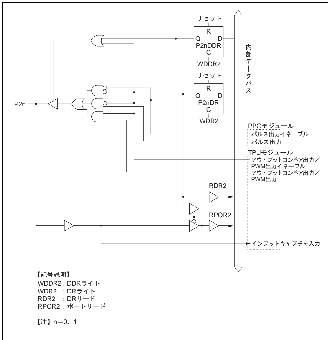
図 C.2 (a) ポート 2 ブロック図 ( P20、 P21 端子 )
