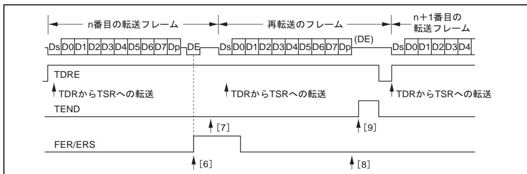
図 15.12 SCI 送信モードの場合の再転送動作
