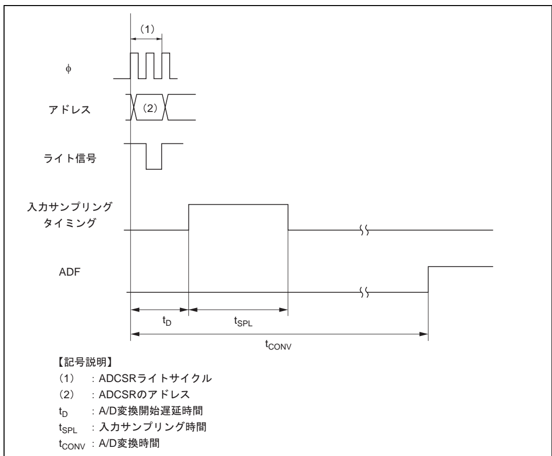
図 16.5 A/D 変換タイミング
