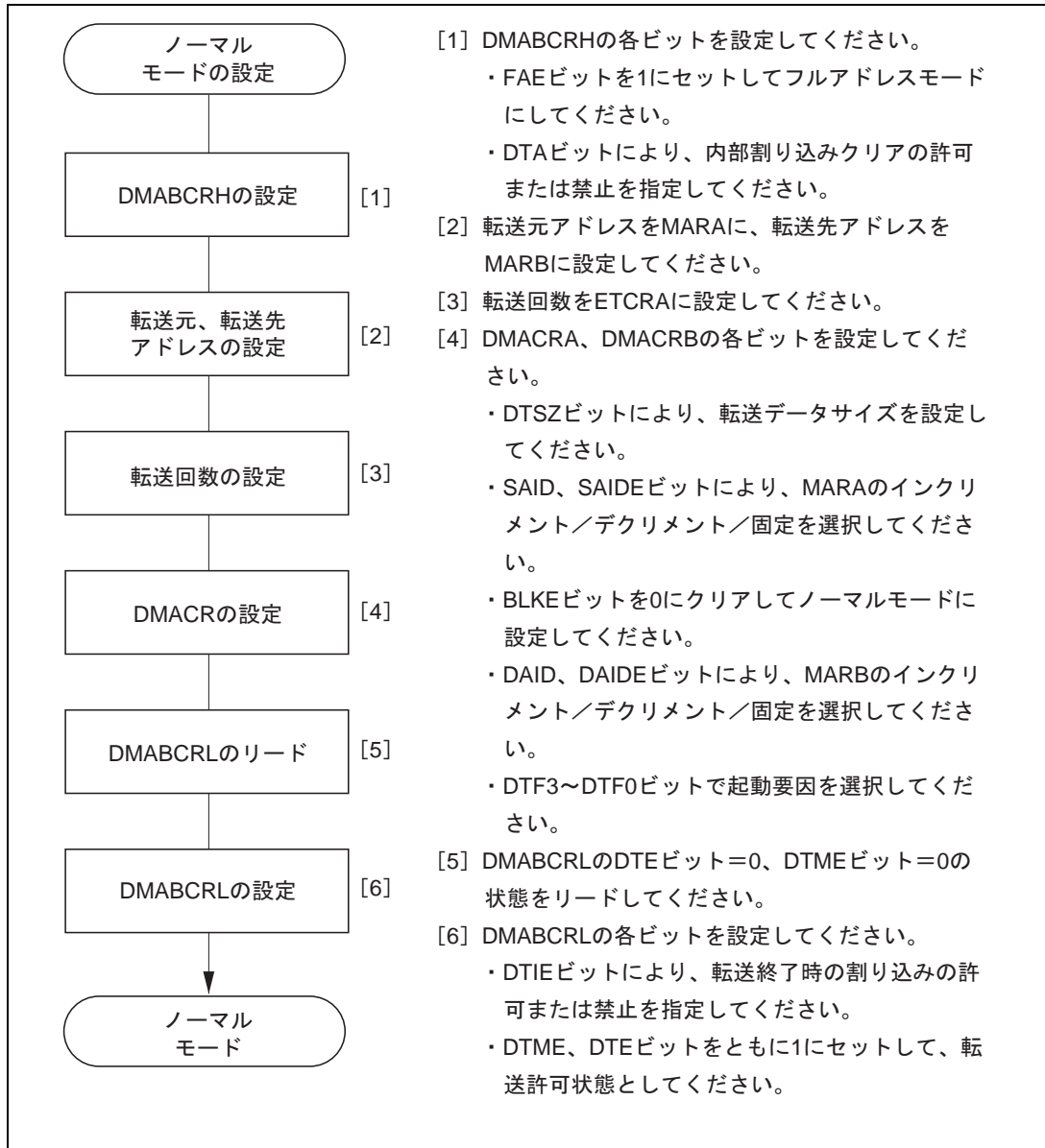
図 7.12 ノーマルモードの設定手順例
