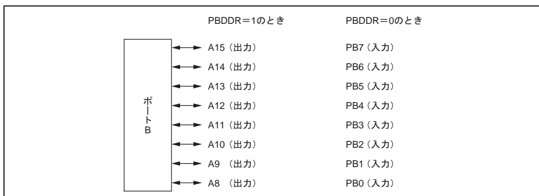
図 9.10 ポート B の端子機能 (モード 6)
