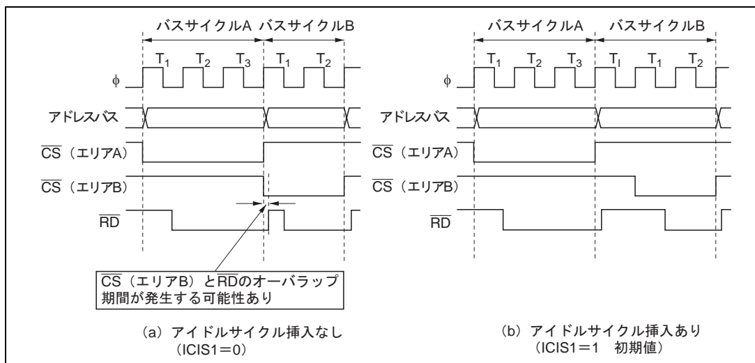
図 6.33 チップセレクト ( \overline{CS} ) とリード ( \overline{RD} ) の関係
