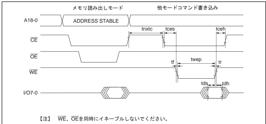
図 19.22 メモリ読み出しモードから他のモードへ遷移時のタイミング波形
