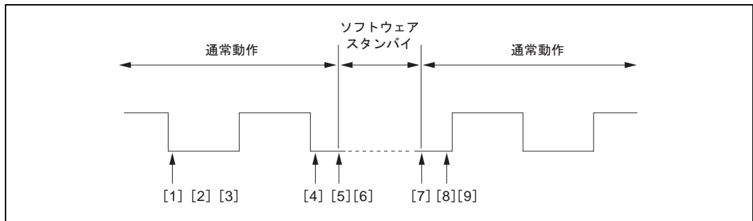
図 15.9 クロック停止・再起動手順
