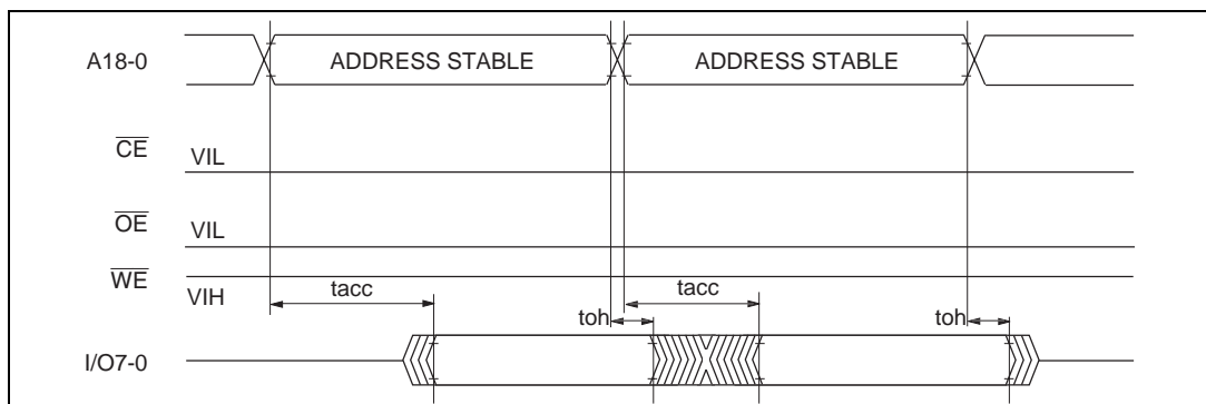
図 19.23 \overline{\text{CE}} 、 \overline{\text{OE}} イネーブル状態リード時のタイミング波形
