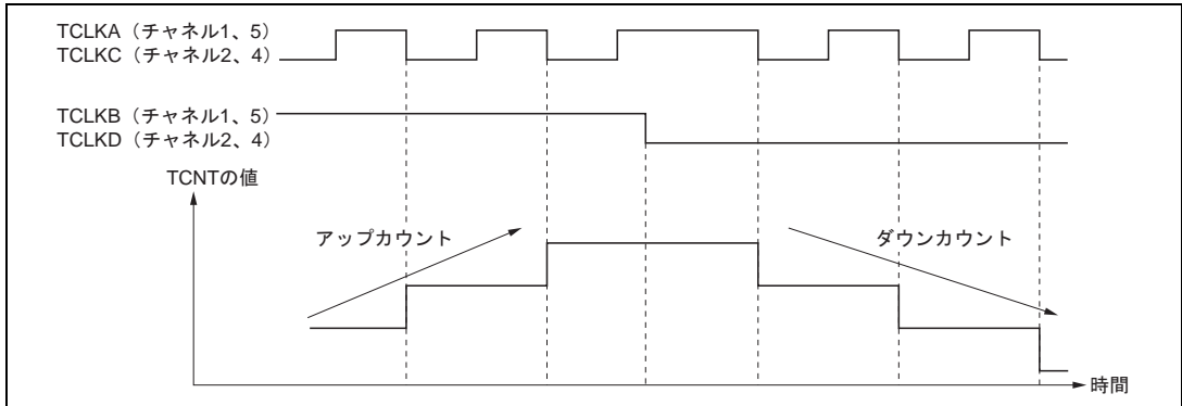
図 10.30 位相計数モード2の動作例
