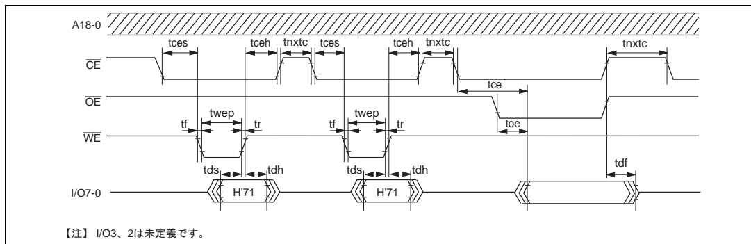
図 19.54 ステータス読み出しモードのタイミング波形
