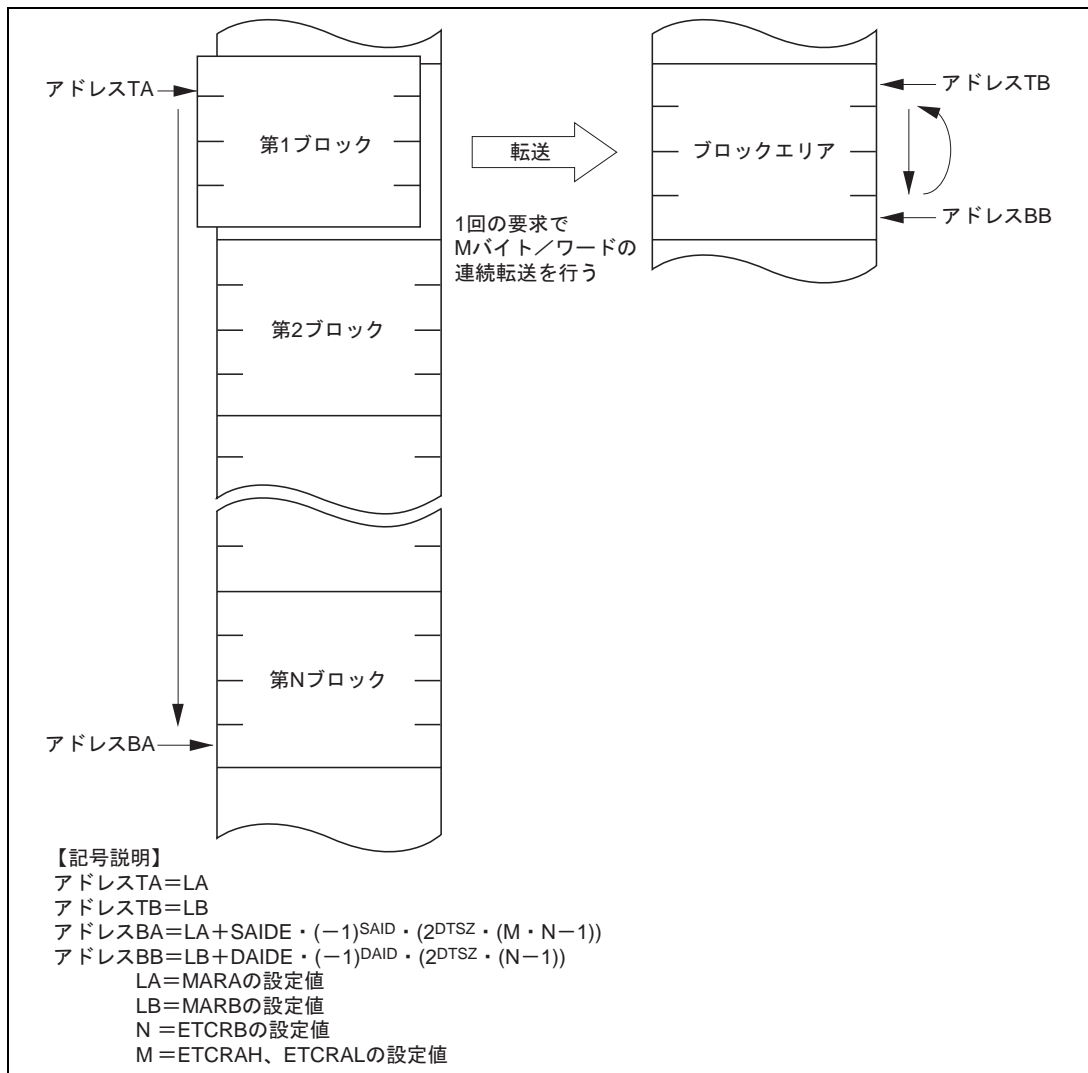
図 7.13 ブロック転送モードの動作 (BLKDIR = 0)
