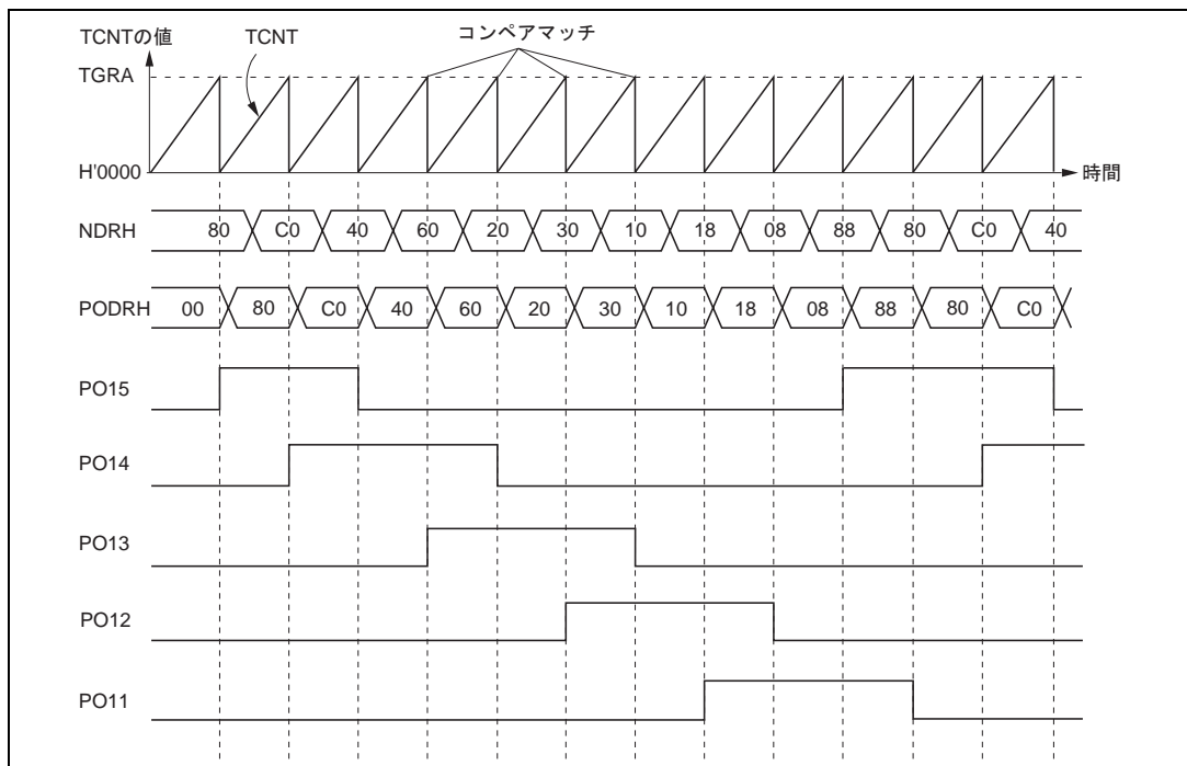
図 11.5 パルス出力通常動作例 (5相パルス出力例)
