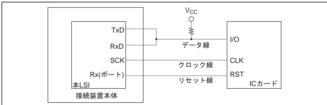
図 15.2 スマートカードインタフェース端子接続概略図
