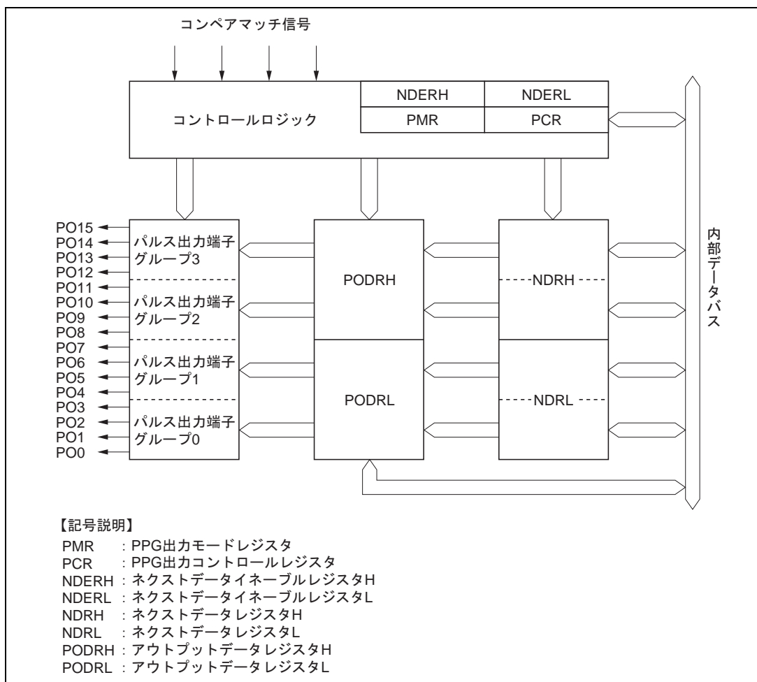
図 11.1 PPGのブロック図
