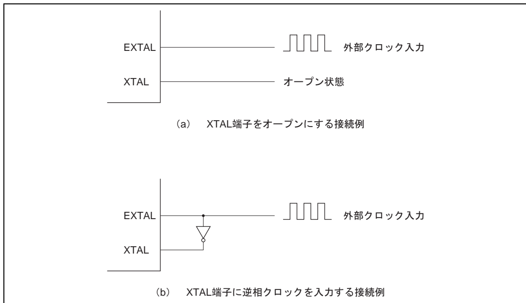
図 20.5 外部クロックの接続例
