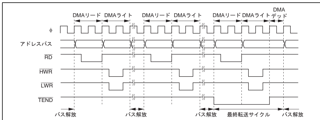
図 7.20 フルアドレスモード (サイクルスチール) 転送例
