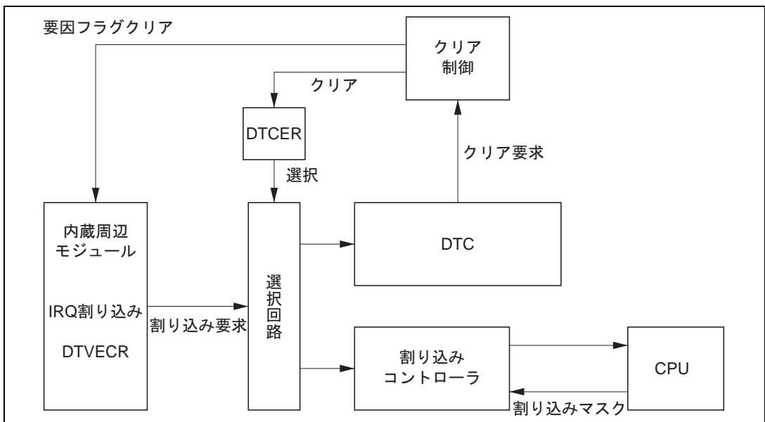
図 8.3 DTC 起動要因制御ブロック図
