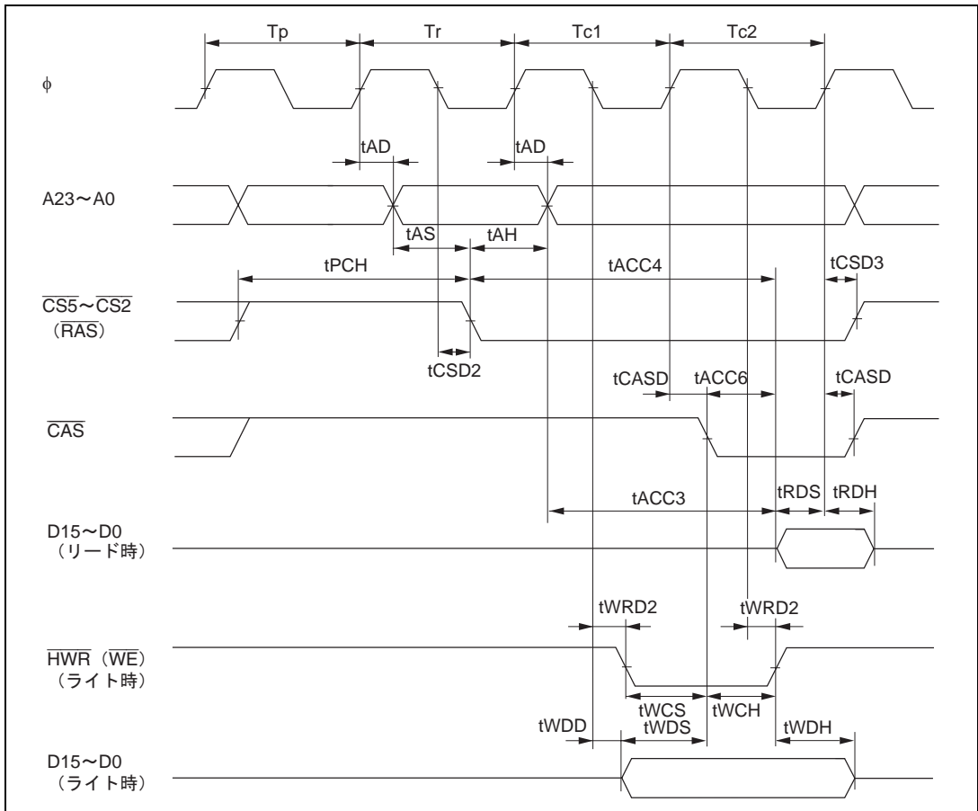
図 22.9 DRAM バスタイミング (H8S/2321 ではサポートされていません)
