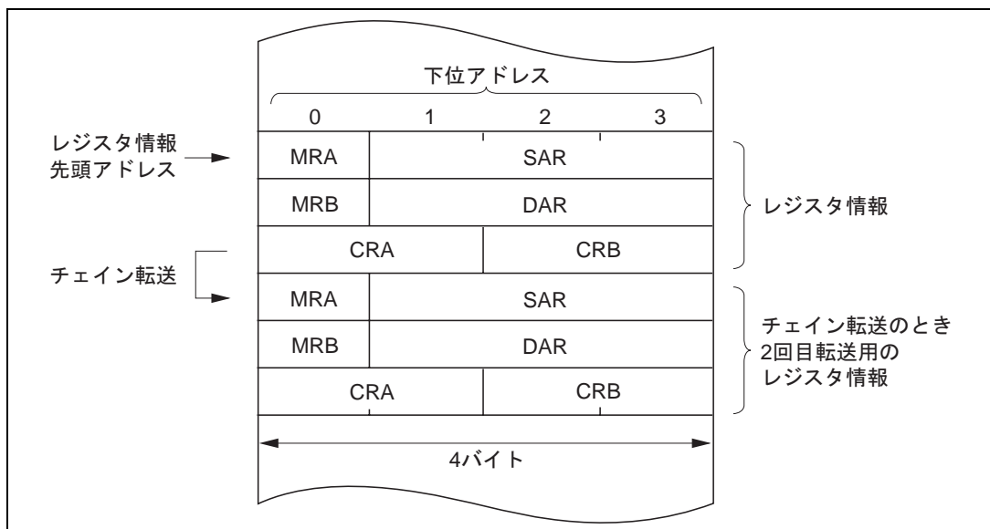
図 8.5 アドレス空間上での DTC レジスタ情報の配置
