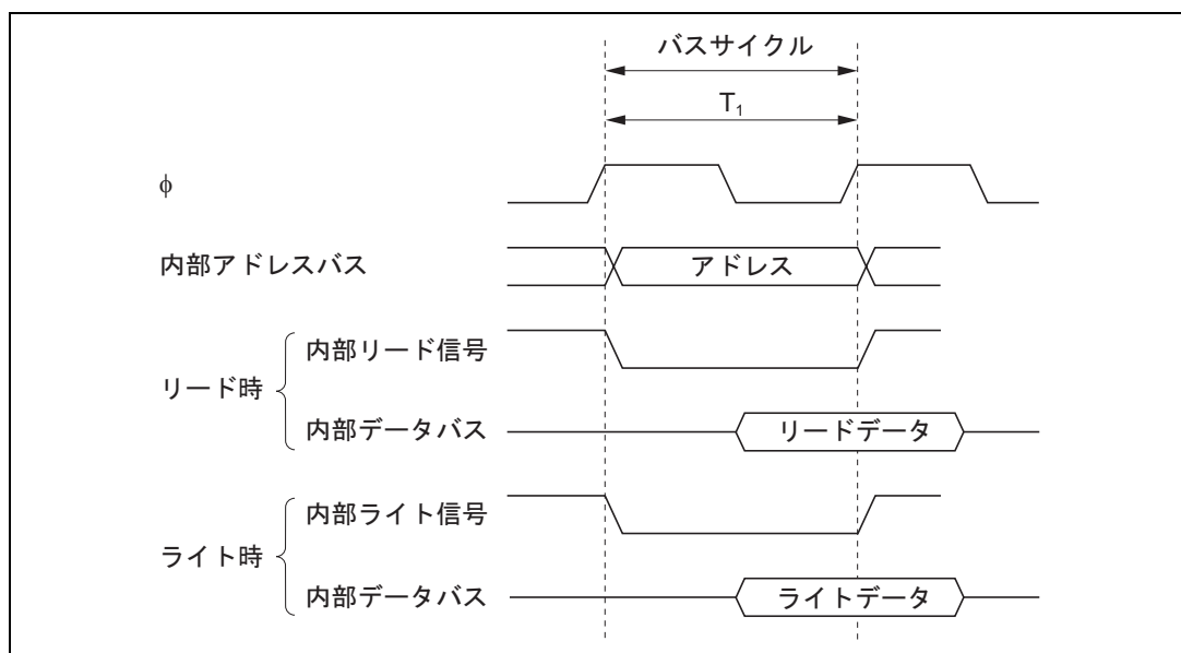
図 2.14 内蔵メモリアクセスサイクル
