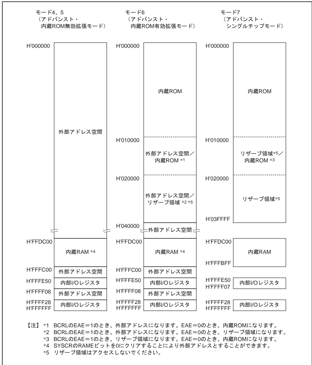
図 3.3 H8S/2327 の各動作モードのアドレスマップ
