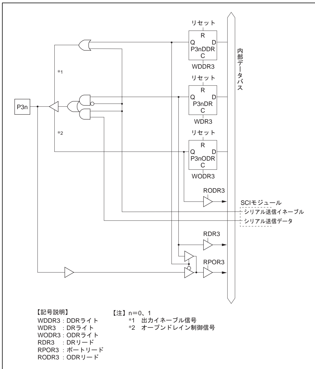
図 C.3 (a) ポート 3 ブロック図 (P30、P31 端子)
