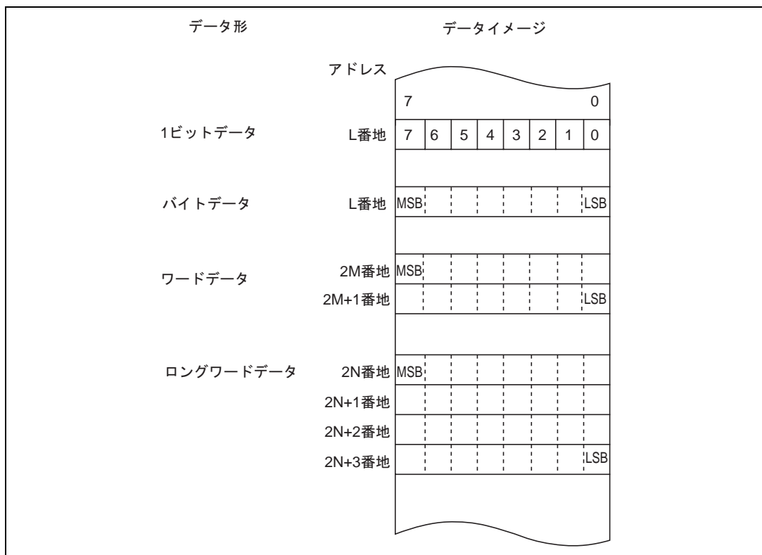
図 2.8 メモリ上でのデータ構成
