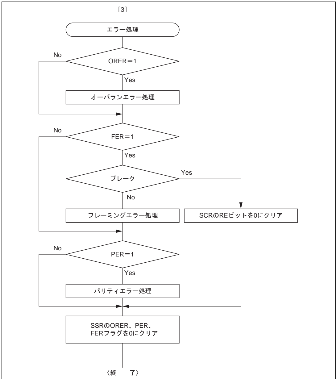
図 14.7 (2) シリアル受信フローチャートの例
