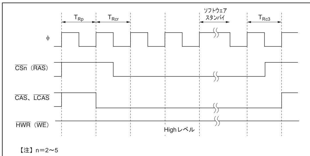
図 6.27 セルフリフレッシュタイミング
