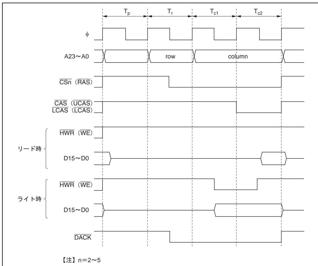
図 6.29 DDS = 0 の場合の \overline{\text{DACK}} 出力タイミング (DRAM アクセスの例)
