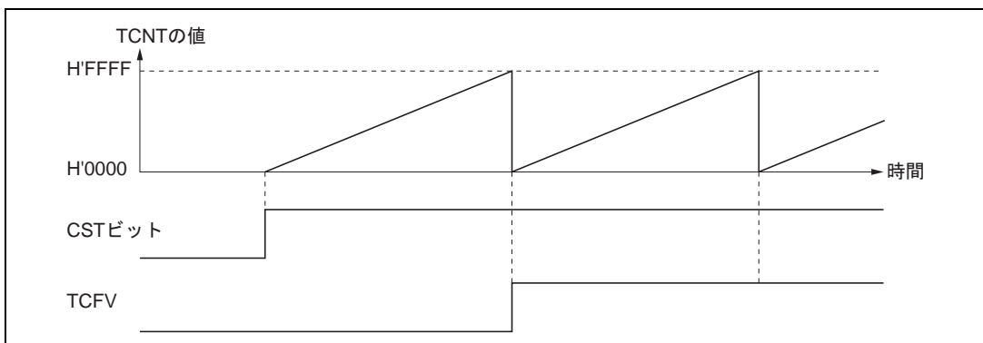
図 10.7 フリーランニングカウンタの動作
