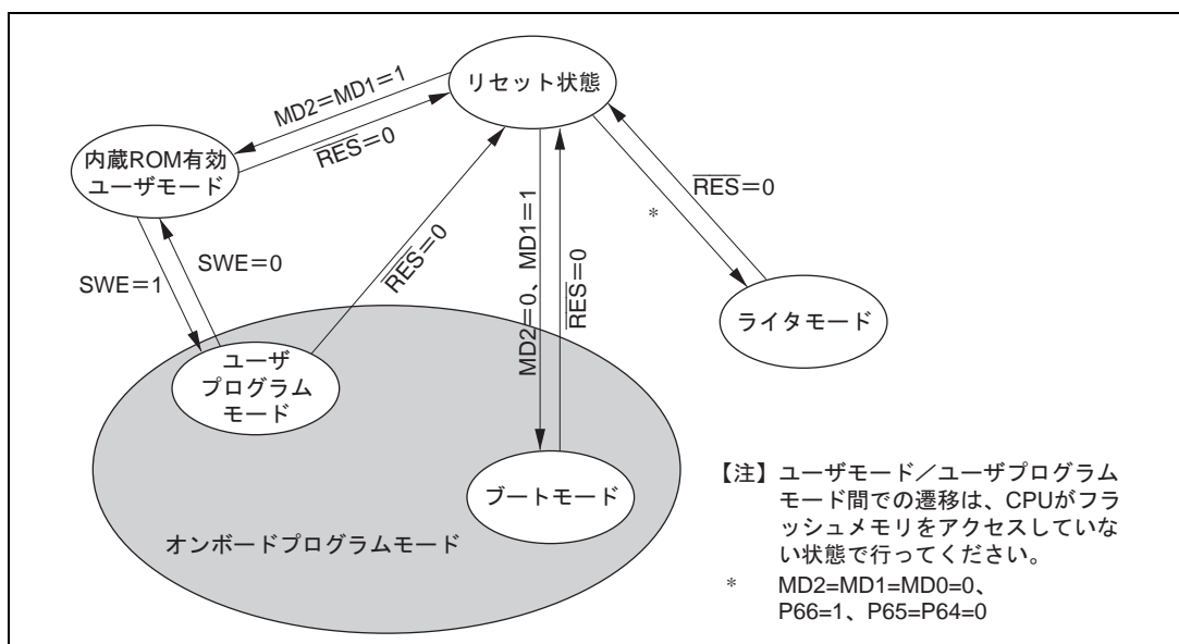
図 19.3 フラッシュメモリに関する状態遷移
