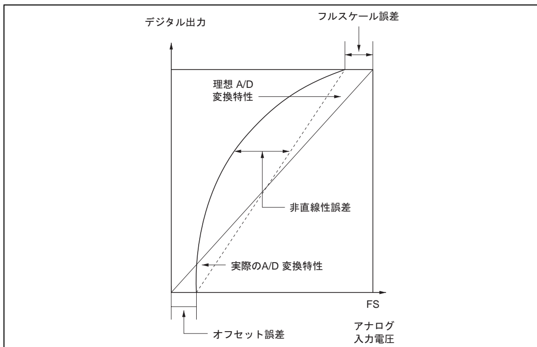
図 16.9 A/D 変換精度の定義 (2)
