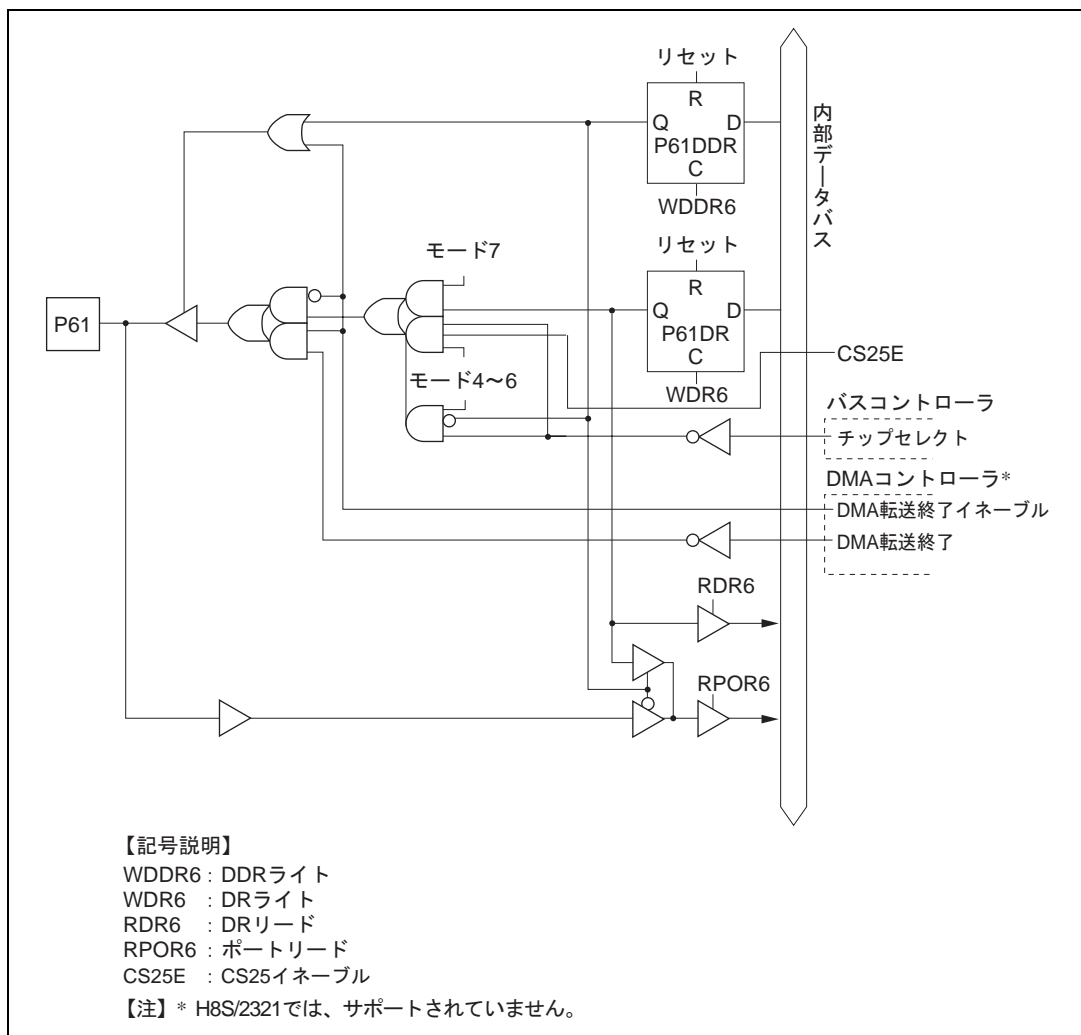
図 C.6 (b) ポート6ブロック図 (P61 端子)
