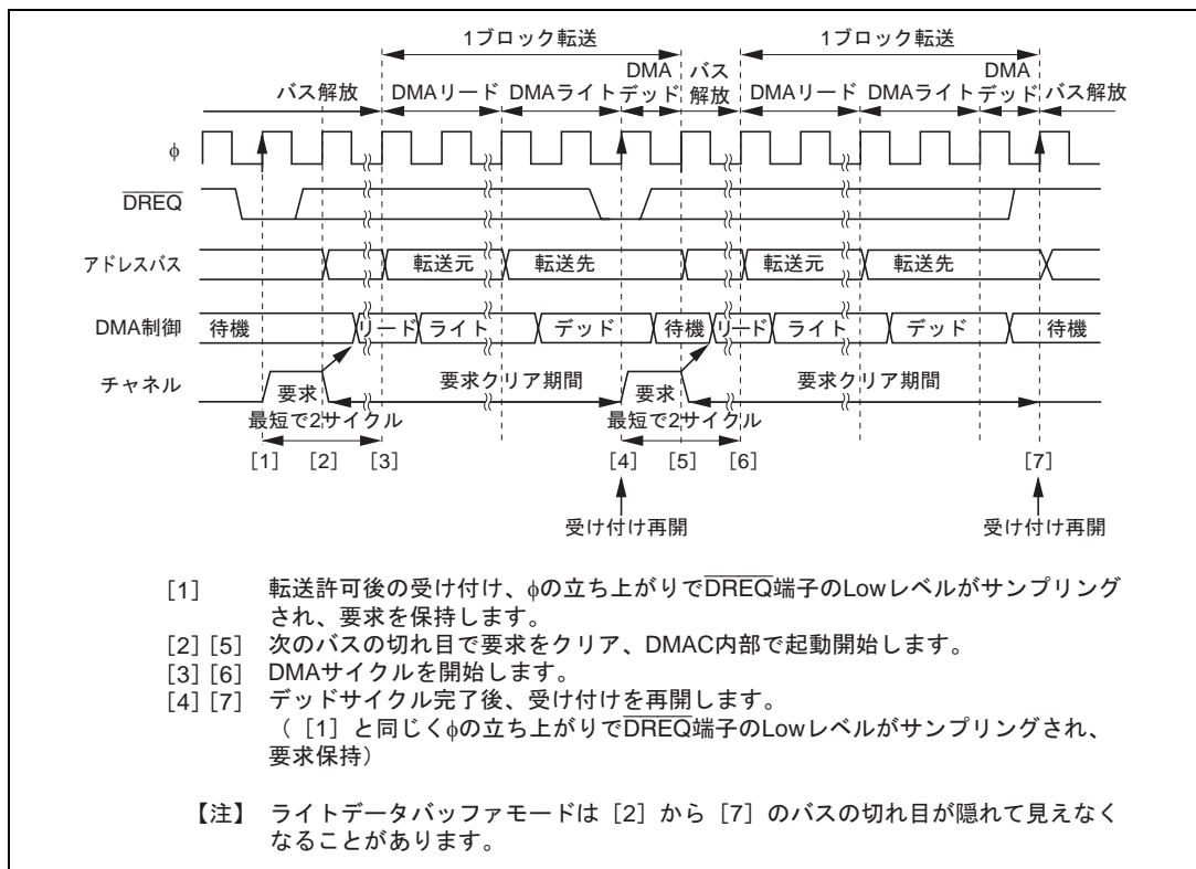
図 7.26 \overline{\text{DREQ}} レベル起動のブロック転送モード転送例
