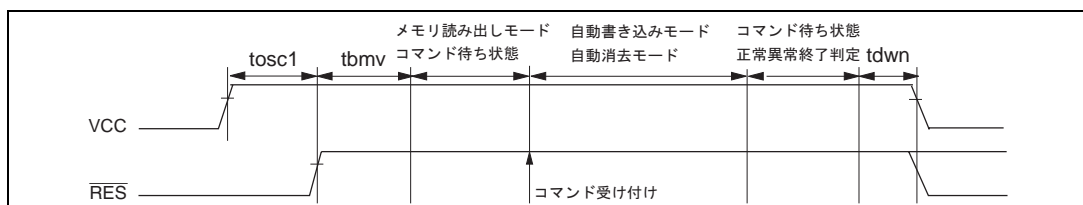
図 19.28 発振安定時間、ライタモードセットアップ、電源立ち下げシーケンス
