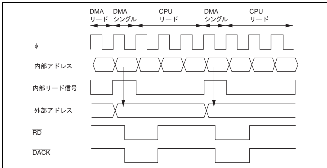
図 7.34 ライトデータバッファ機能を用いたシングルアドレス転送の例
