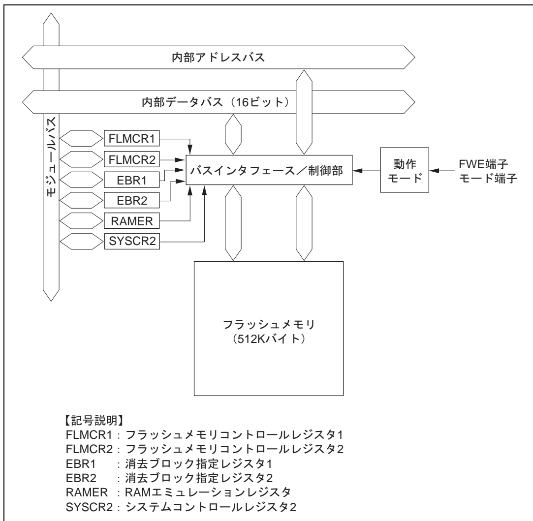
図 19.59 フラッシュメモリのブロック図
