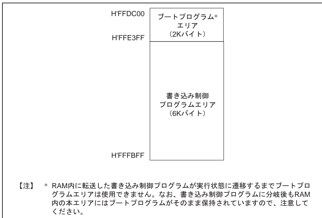
図 19.39 ブートモード時の RAM エリア
