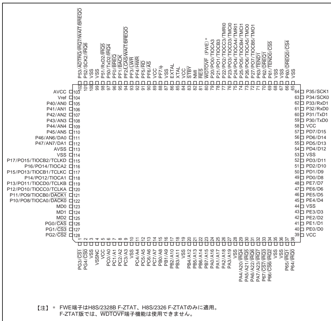
図 1.4 マスク ROM 版、F-ZTAT 版、H8S/2324S、H8S/2322R、H8S/2320 ピン配置図 (FP-128B : 上面図)
