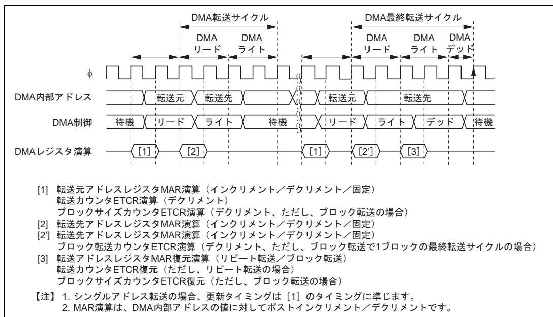
図 7.40 DMAC レジスタの更新タイミング
