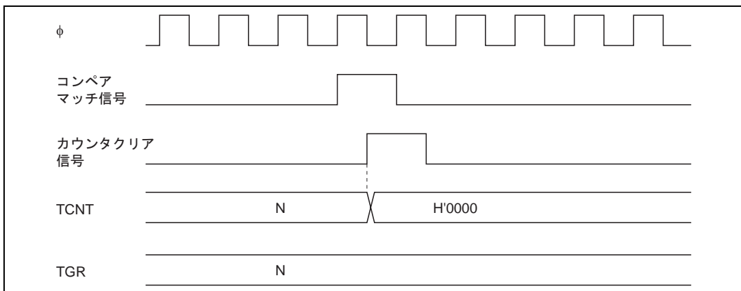
図 10.38 カウンタクリアタイミング (コンペアマッチ)
