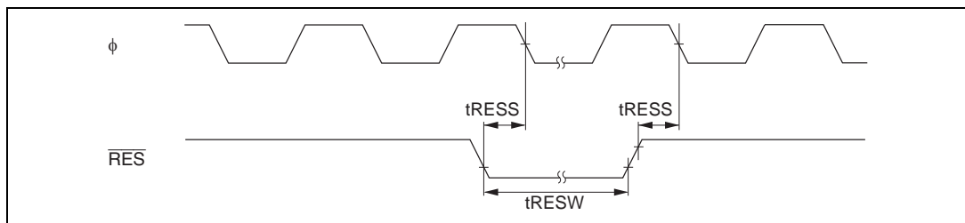
図 22.4 リセット入力タイミング
