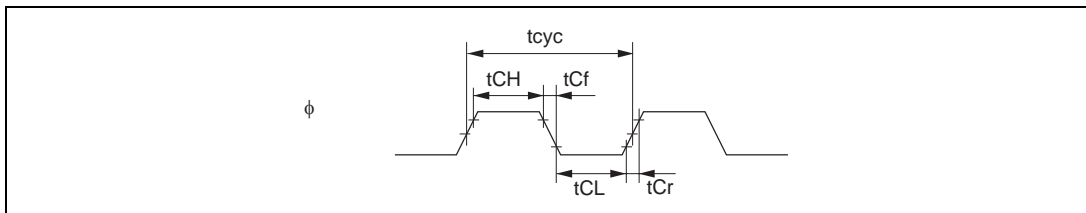
図 22.2 システムクロックタイミング
