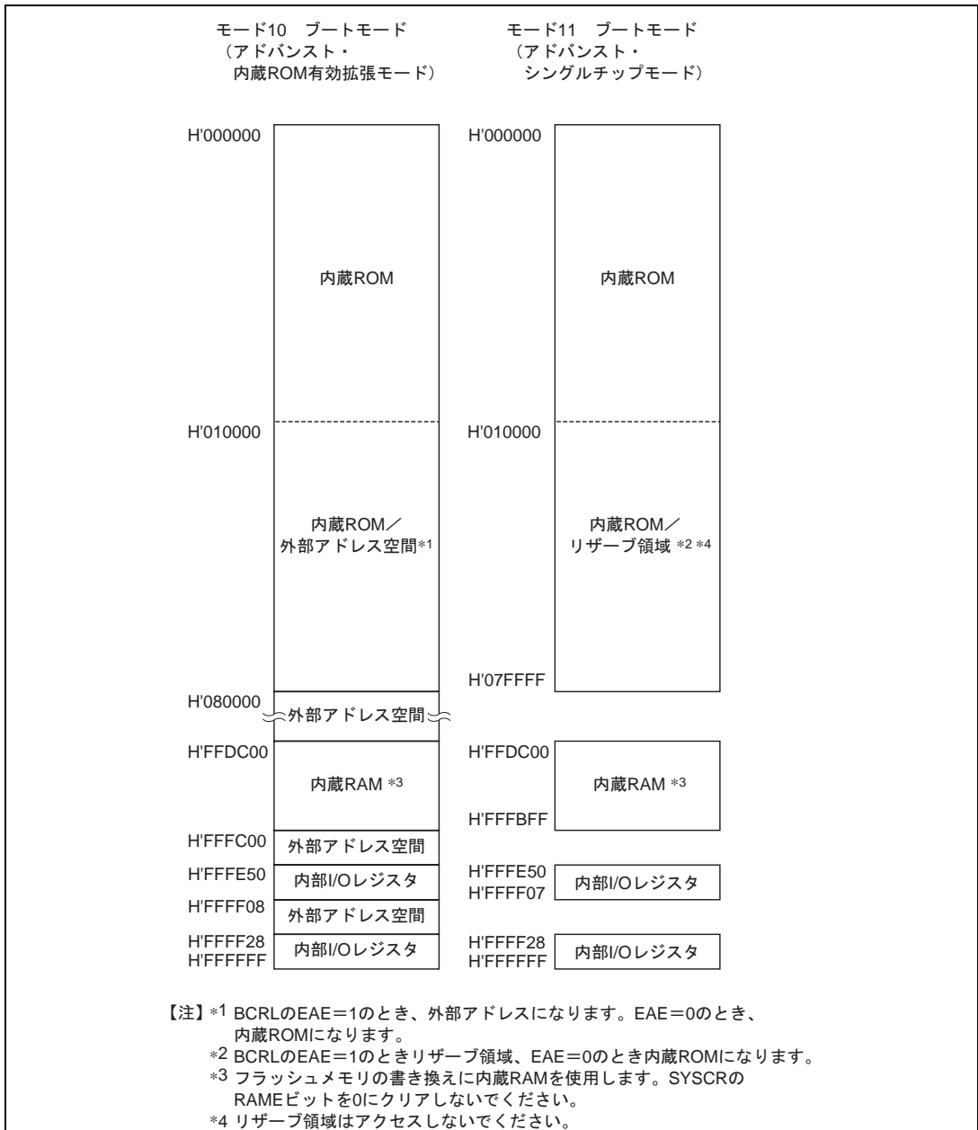
図 3.4 H8S/2326 F-ZTAT の各動作モードのアドレスマップ (2)
