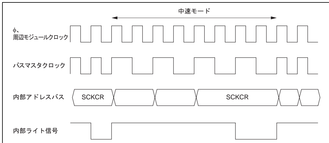
図 21.1 中速モードの遷移・解除タイミング
