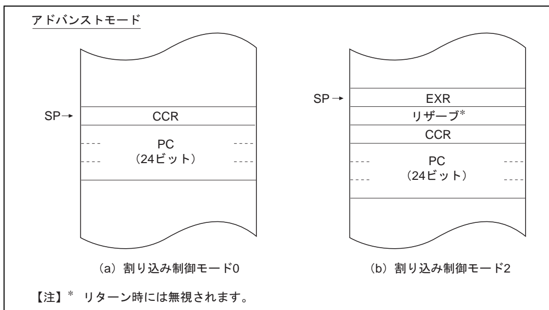
図 2.13 例外処理終了後のスタックの状態 (例)
