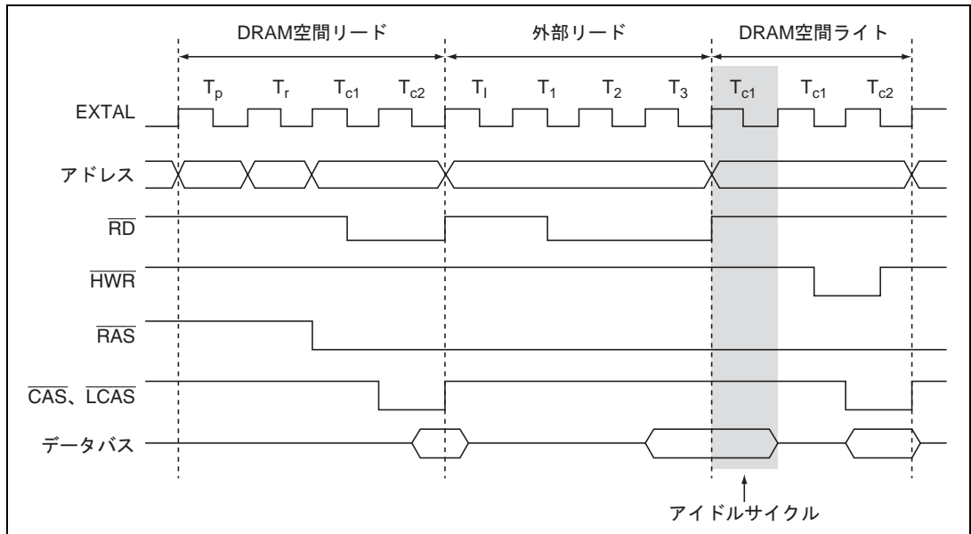
図 6.35 (b) RAS ダウンモード時のアイドルサイクル動作例 (ICIS0 = 1)
