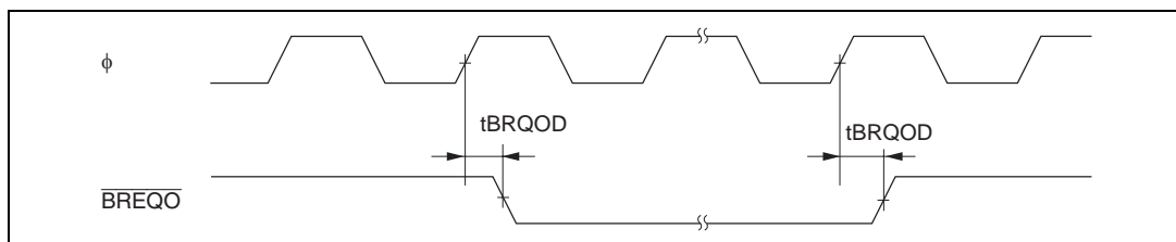
図 22.15 外部バス権要求出力タイミング
