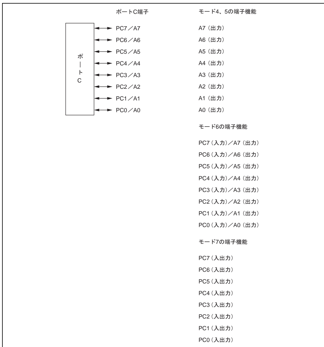
図 9.12 ポート C の端子機能
