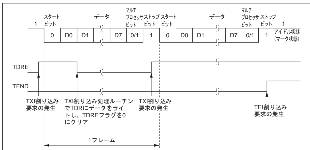
図 14.11 SCI の送信時の動作例 (8ビットデータ/マルチプロセッサビットあり/1ストップビットの例)
