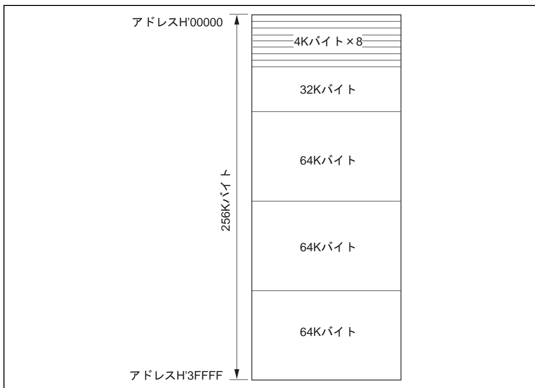
図 19.35 ブロック分割法
