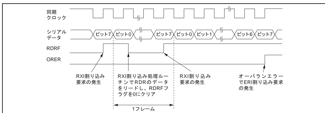
図 14.19 SCI の受信時の動作例
