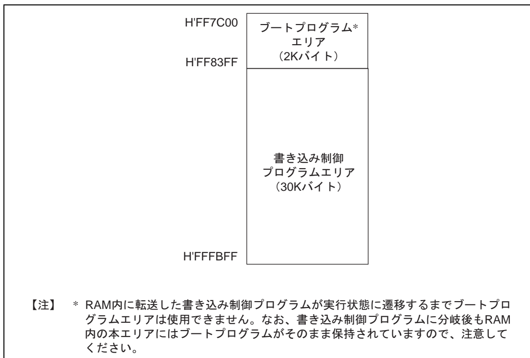
図 19.12 ブートモード時の RAM エリア
