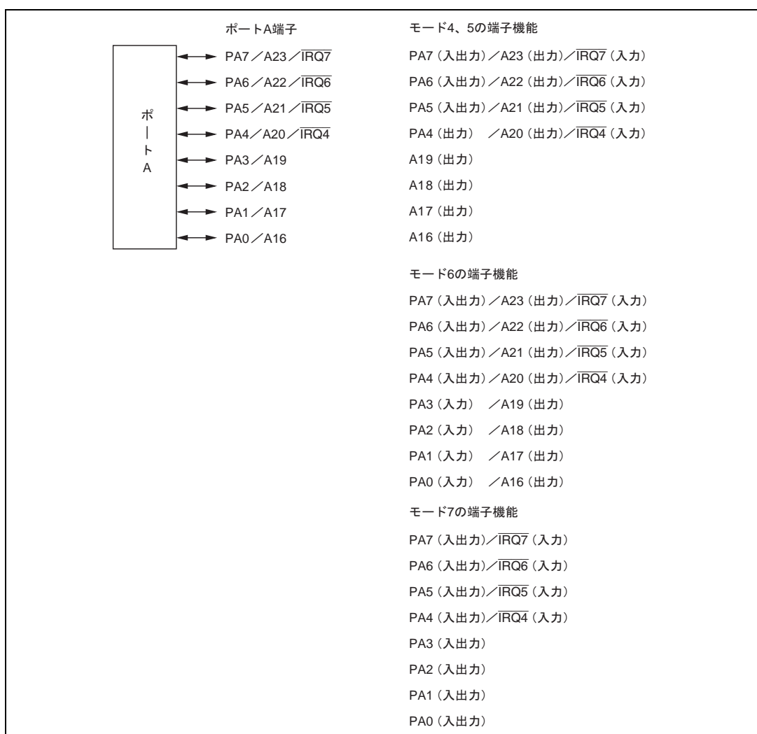
図 9.7 ポート A の端子機能
