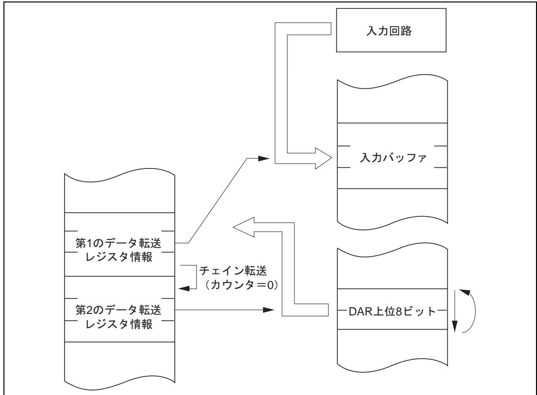
図 8.13 カウンタ=0時のチェーン転送
