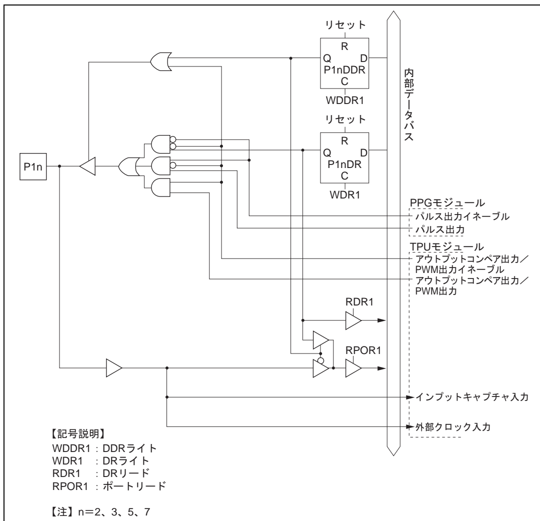
図 C.1 (b) ポート 1 ブロック図 (P12、P13、P15、P17 端子)
