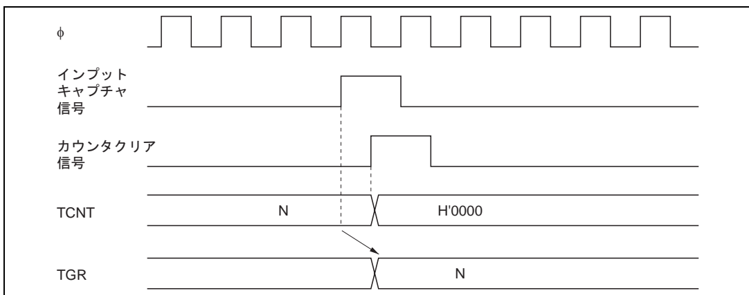
図 10.39 カウンタクリアタイミング (インプットキャプチャ)
