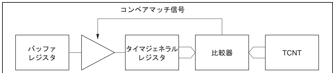
図 10.16 コンペアマッチバッファ動作
