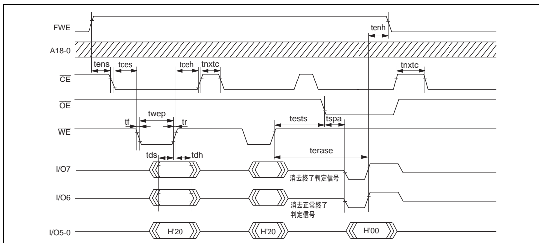
図 19.83 自動消去モードのタイミング波形
