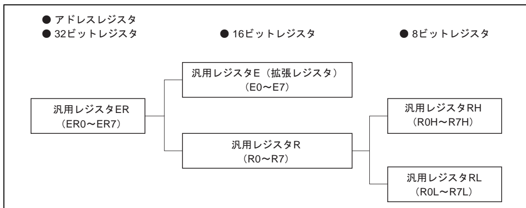
図 2.5 汎用レジスタの使用方法
