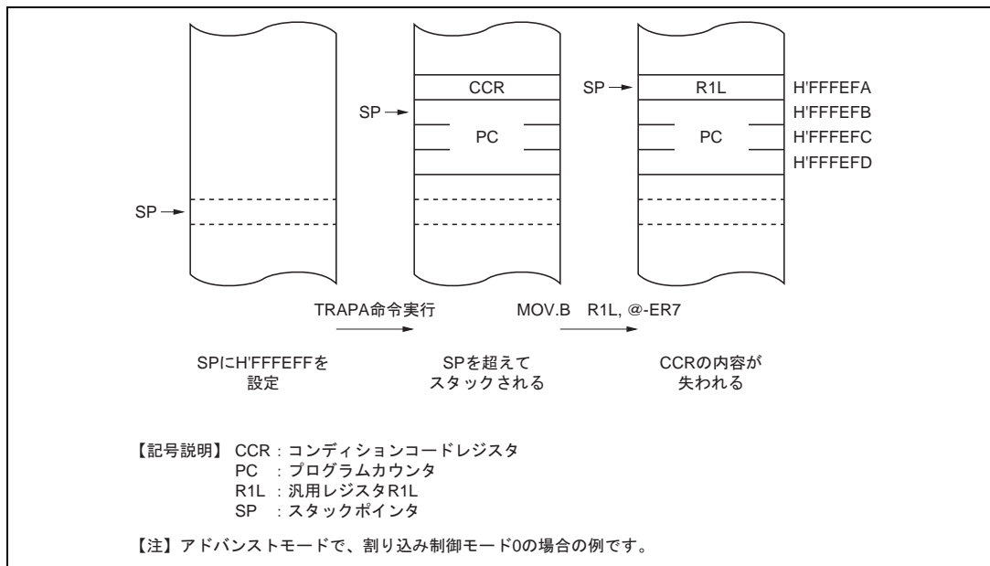
図 4.5 SP を奇数に設定したときの動作
