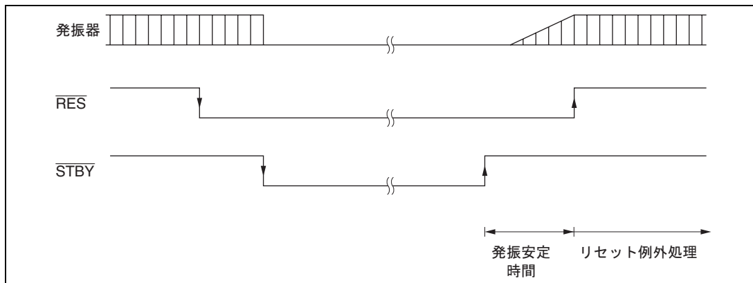
図 21.3 ハードウェアスタンバイモードのタイミング
