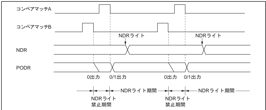
図 11.11 ノンオーバーラップ動作と NDR ライトタイミング
