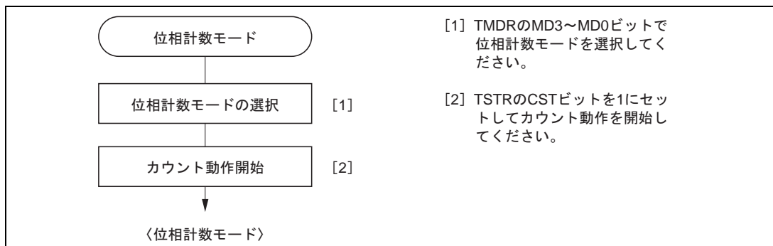
図 10.28 位相計数モードの設定手順例
