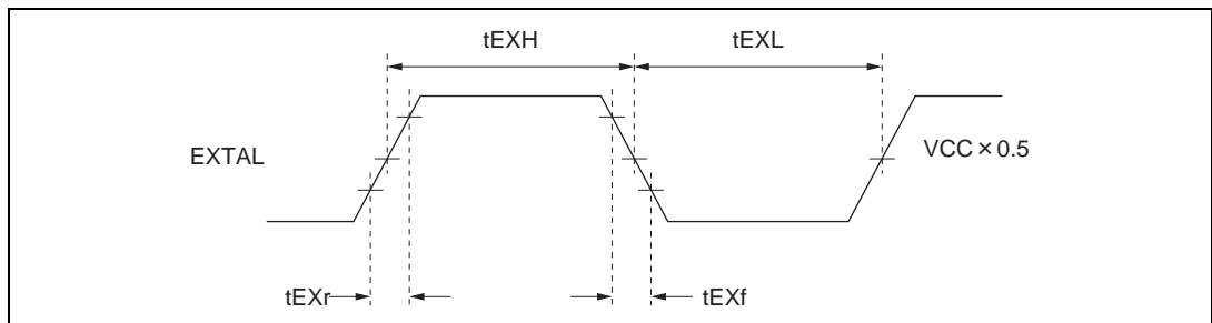
図 20.6 外部クロック入力タイミング
