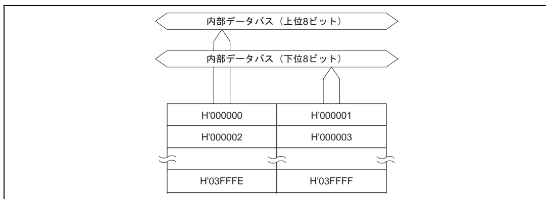
図 19.1 ROM のブロック図 (256K バイト)
