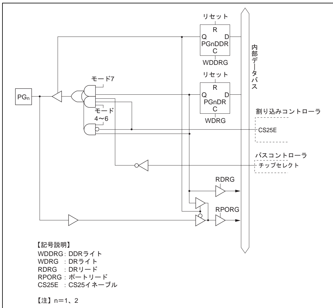
図 C.13 (b) ポート G ブロック図 (PG1、PG2 端子)
