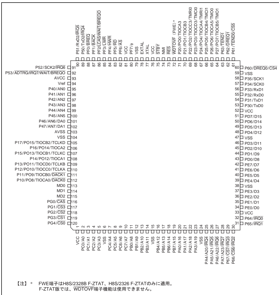
図 1.3 マスク ROM 版、F-ZTAT 版、H8S/2324S、H8S/2322R、H8S/2320 ピン配置図 (TFP-120：上面図)
