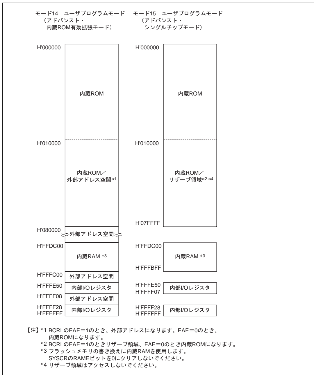
図 3.4 H8S/2326 F-ZTAT の各動作モードのアドレスマップ (3)
