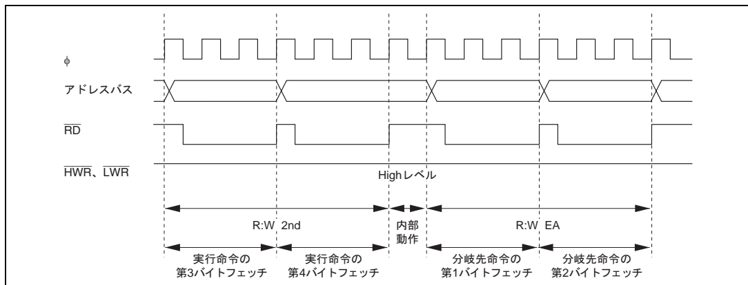
図 A.1 アドレスバス、RD、HWR、LWRのタイミング (8ビットバス・3ステートアクセス・ウェイトなしの場合)
