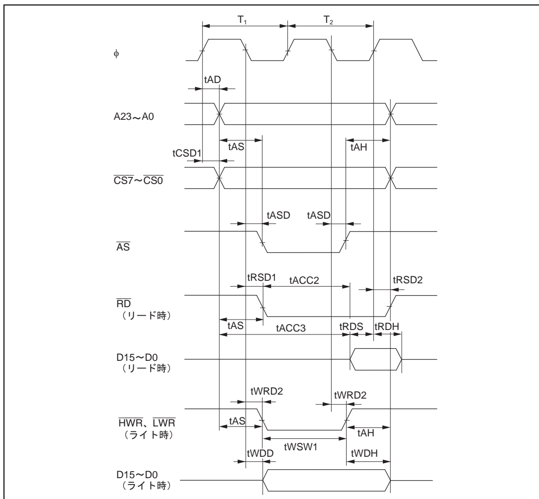
図 22.6 基本バスタイミング / 2 ステートアクセス
