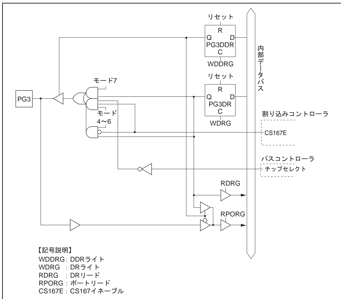
図 C.13 (c) ポート G ブロック図 (PG3 端子)
