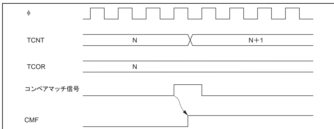
図 12.4 CMF セットタイミング
