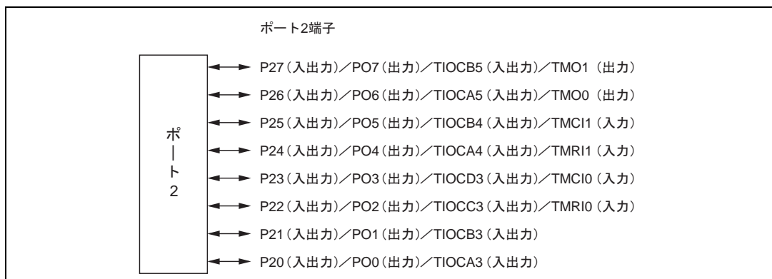
図 9.2 ポート 2 の端子機能
