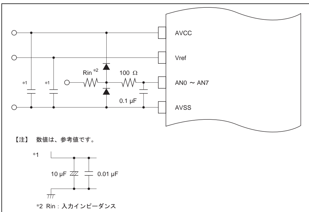
図 16.7 アナログ入力保護回路の例
