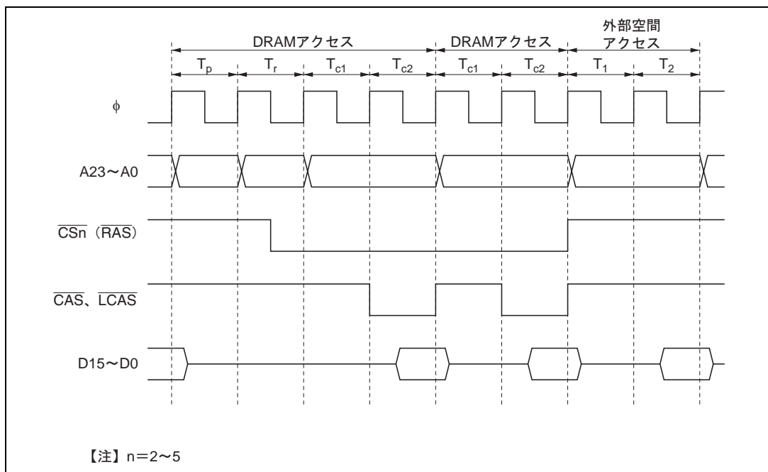
図 6.22 RAS アップモードの動作タイミング例
