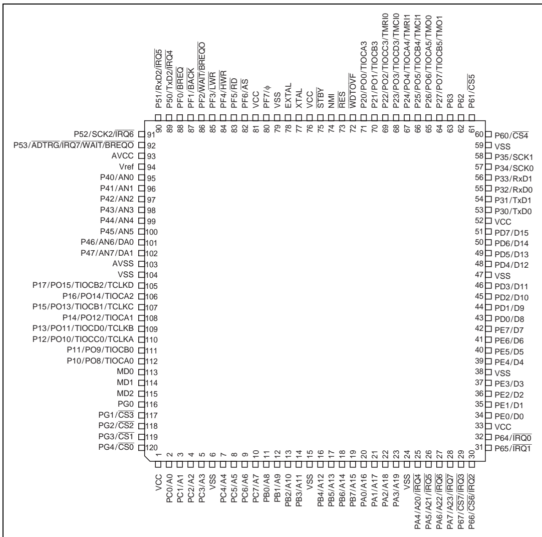
図 1.5 H8S/2321 ピン配置図 (TFP-120 : 上面図)
