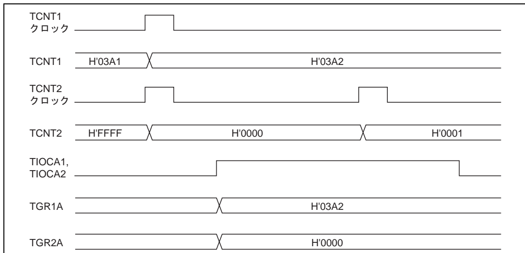
図 10.22 カスケード接続動作例 (1)
