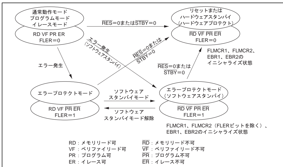
図 19.16 フラッシュメモリの状態遷移図
