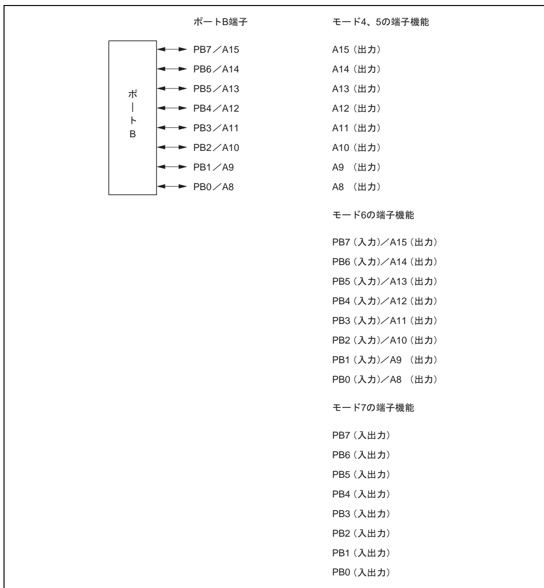
図 9.8 ポート B の端子機能
