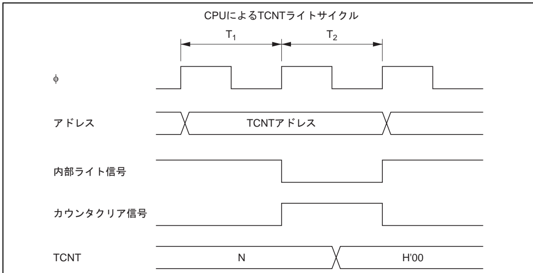
図 12.10 TCNTのライトとクリアの競合
