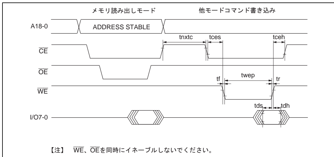
図 19.49 メモリ読み出しモードから他のモードへ遷移時のタイミング波形
