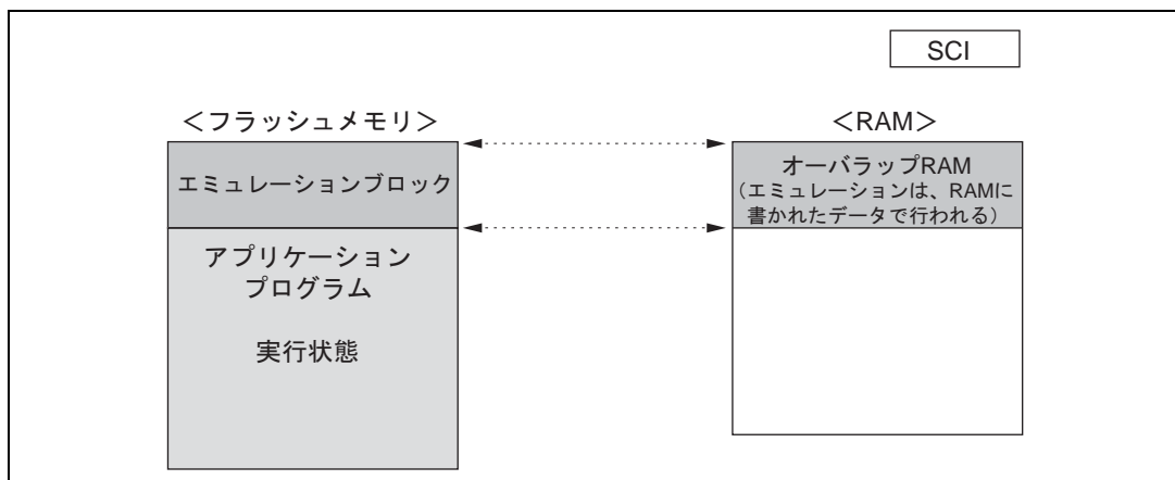
図 19.6 ユーザモード、ユーザプログラムモードのオーバーラップ RAM データの読み出し
