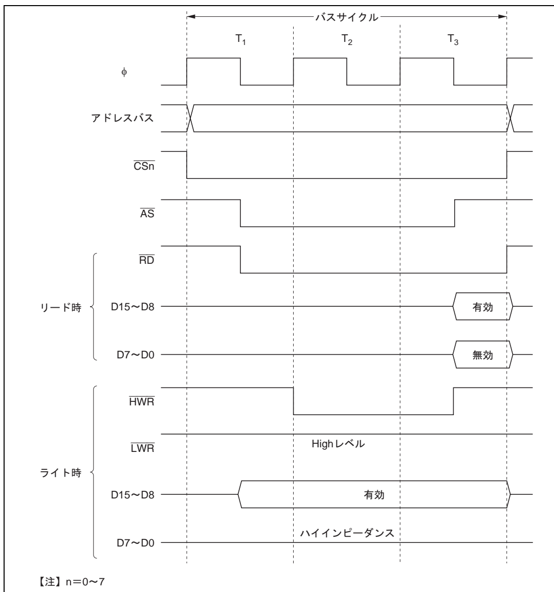
図 6.7 8 ビット 3 ステートアクセス空間のバスタイミング
