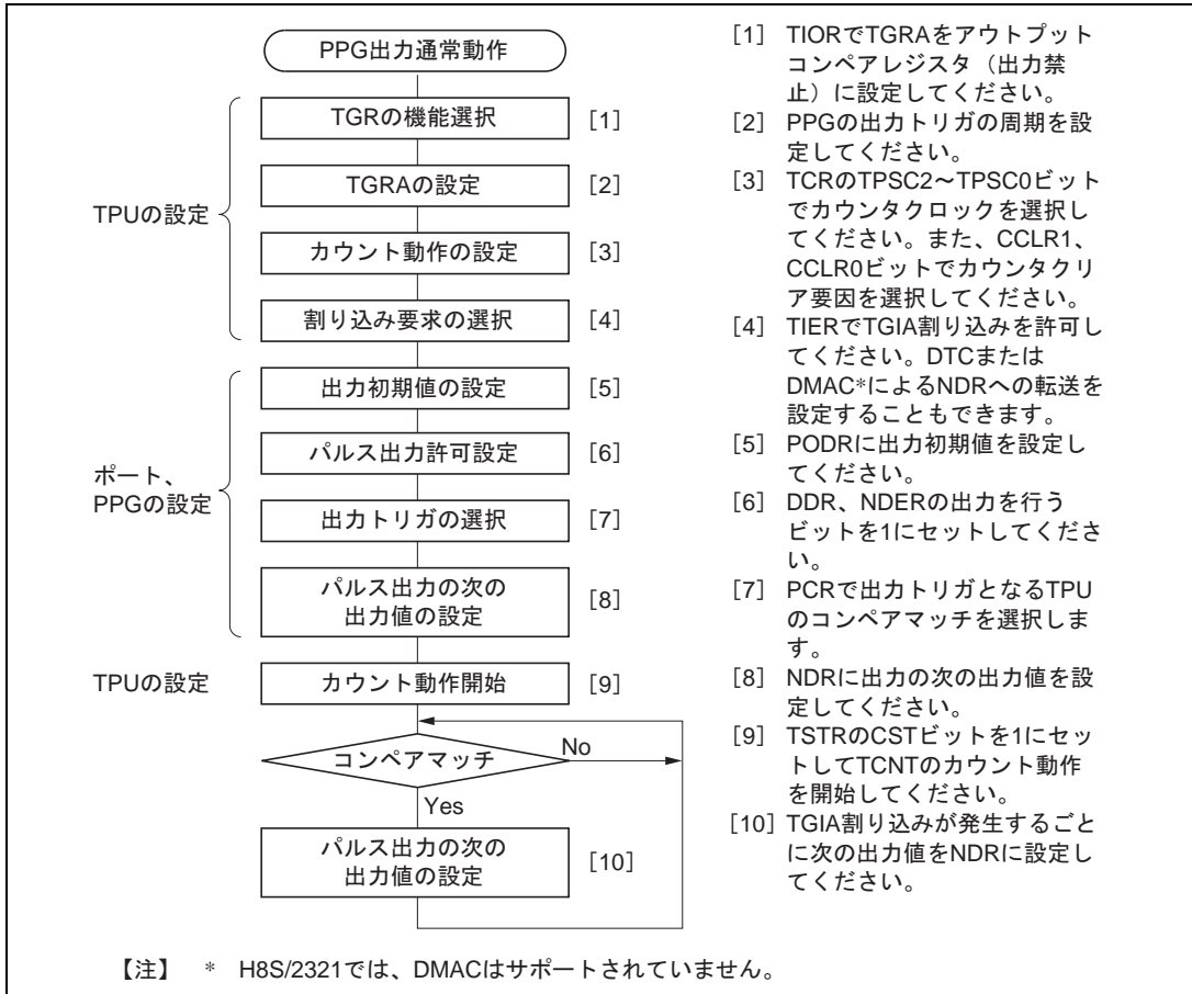
図 11.4 パルス出力通常動作の設定手順例
