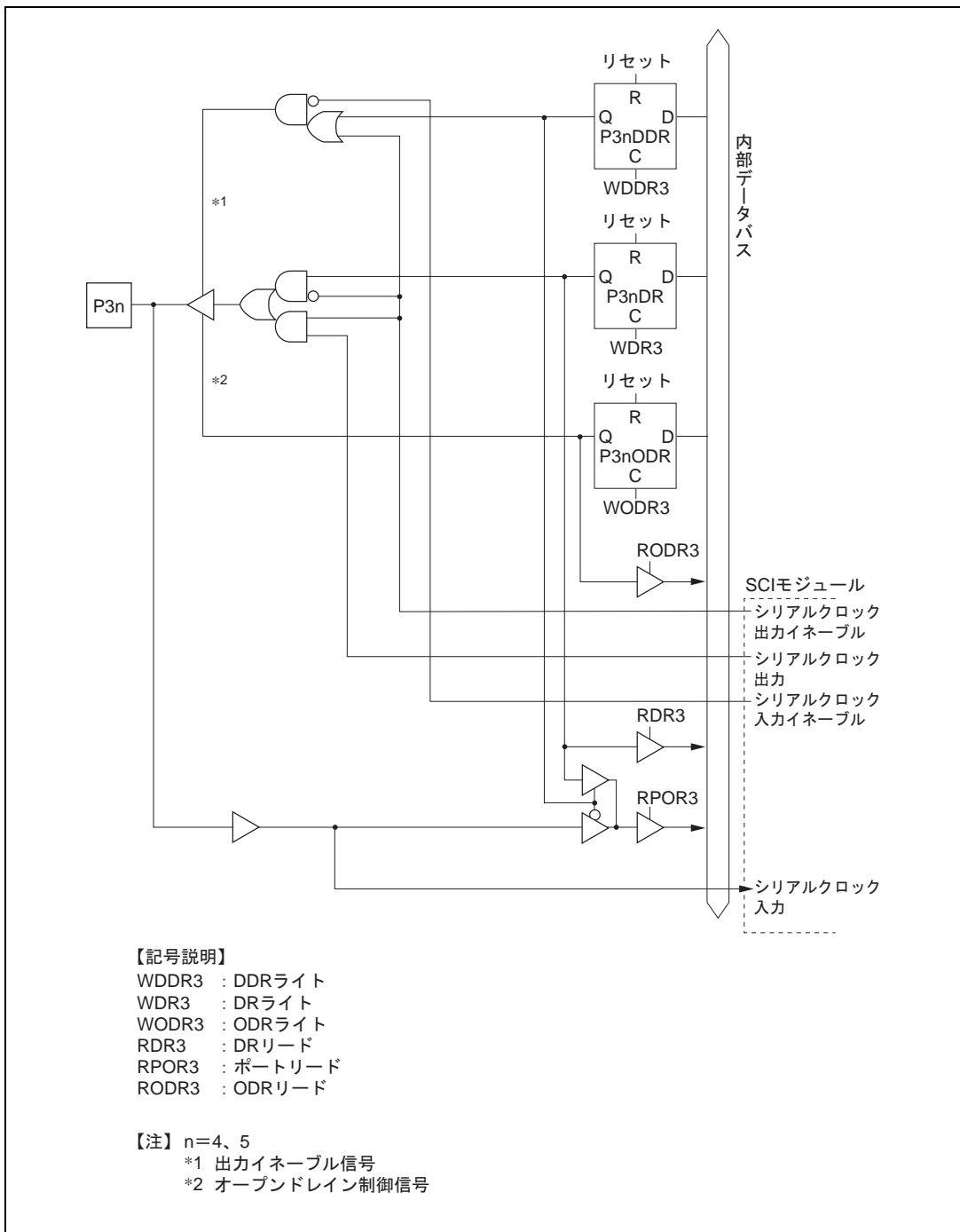
図 C.3 (c) ポート 3 ブロック図 (P34、P35 端子)
