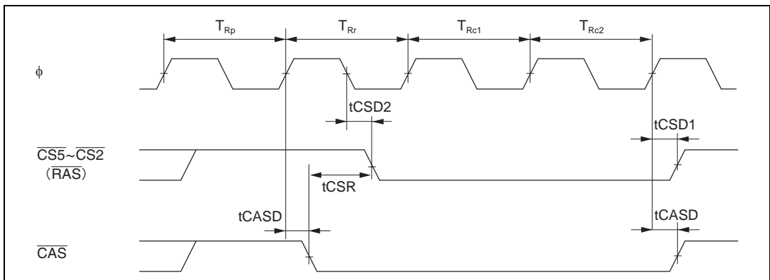
図 22.10 CAS ビフォ RAS リフレッシュタイミング (H8S/2321 ではサポートされていません)
