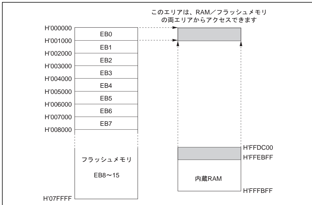
図 19.75 RAM のオーバーラップ動作例
