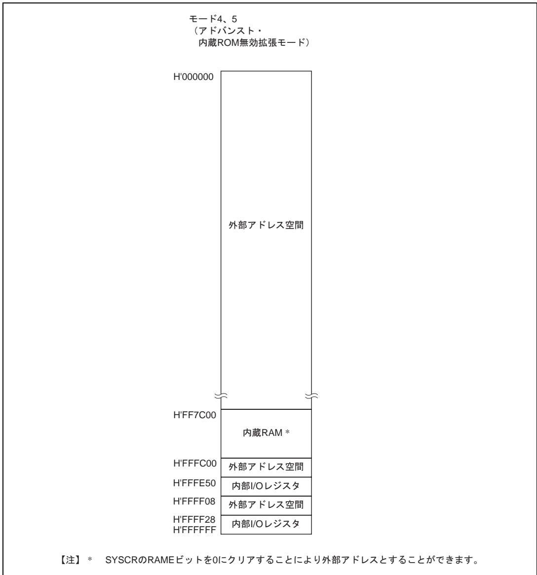
図 3.5 H8S/2324S の各動作モードのアドレスマップ
