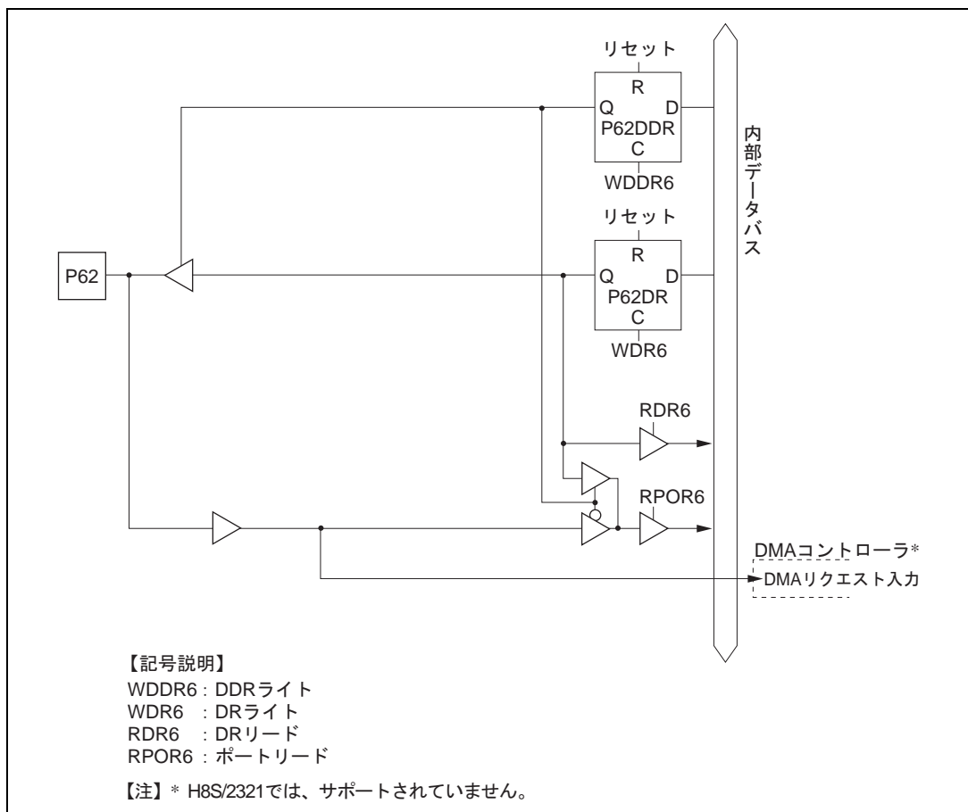
図 C.6 (c) ポート 6 ブロック図 (P62 端子)
