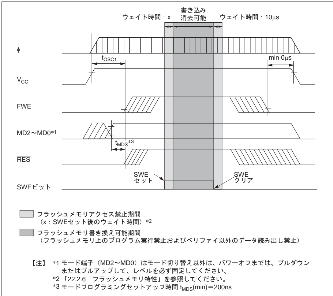
図 19.57 電源投入/切断タイミング (ユーザプログラムモード)
