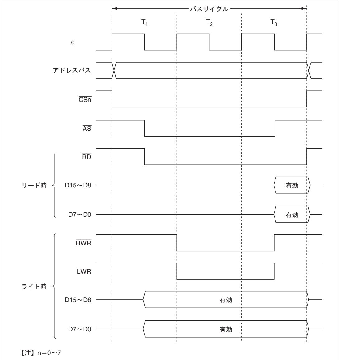
図 6.13 16 ビット 3 ステートアクセス空間のバスタイミング (3) (ワードアクセス)
