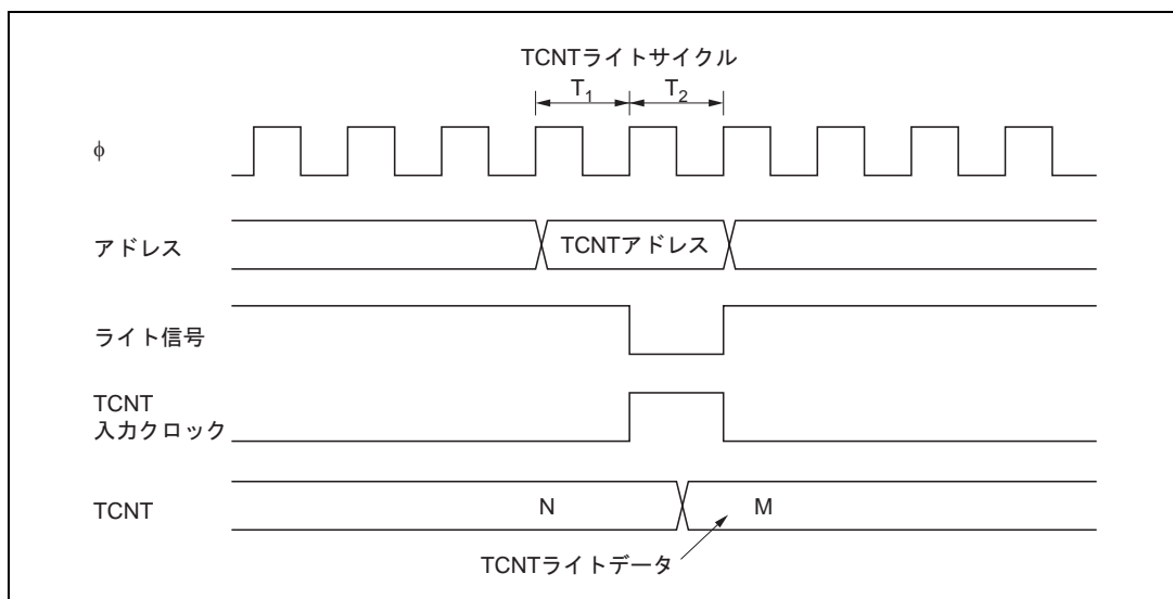
図 10.50 TCNT のライトとカウントアップの競合
