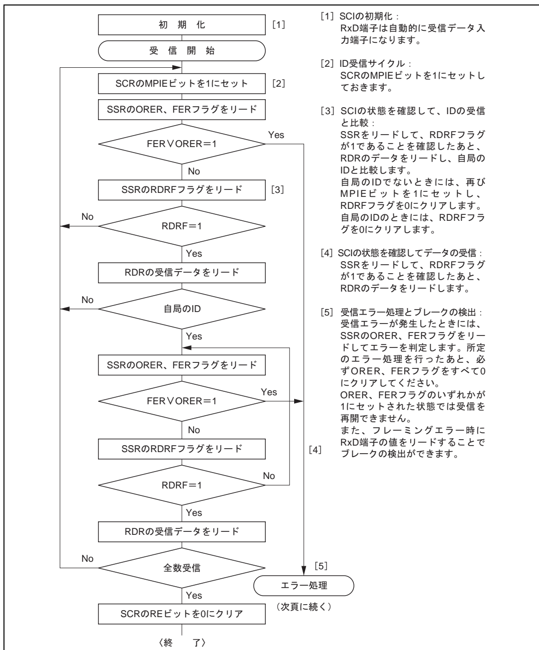
図 14.12 (1) マルチプロセッサシリアル受信フローチャートの例
