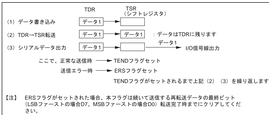
図 15.5 送信動作と内部レジスタの関連
