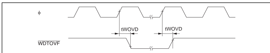
図 22.27 WDT 出力タイミング
