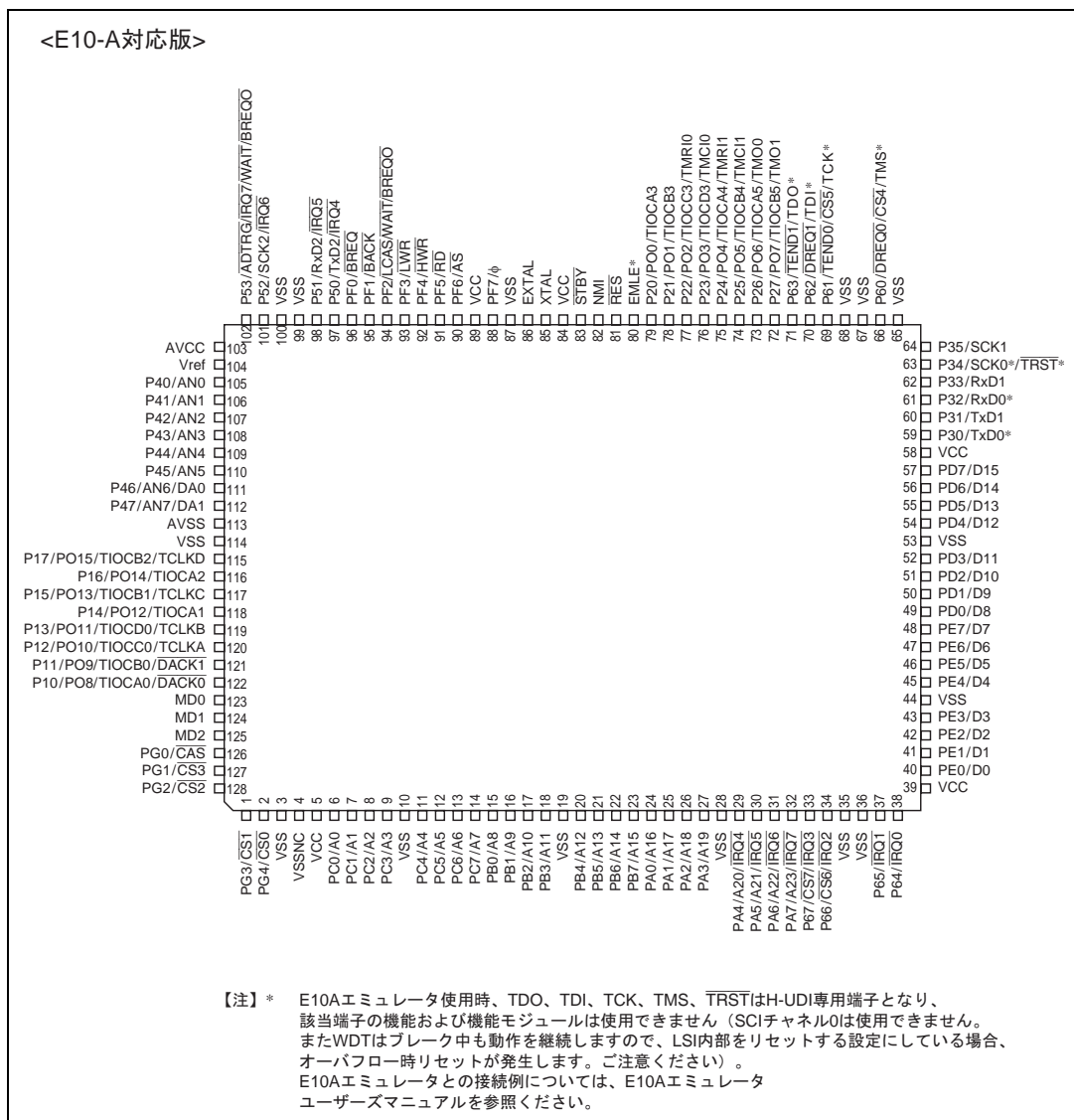
図 1.10 HD64F2329E ピン配置図 (FP-128B : 上面図)
