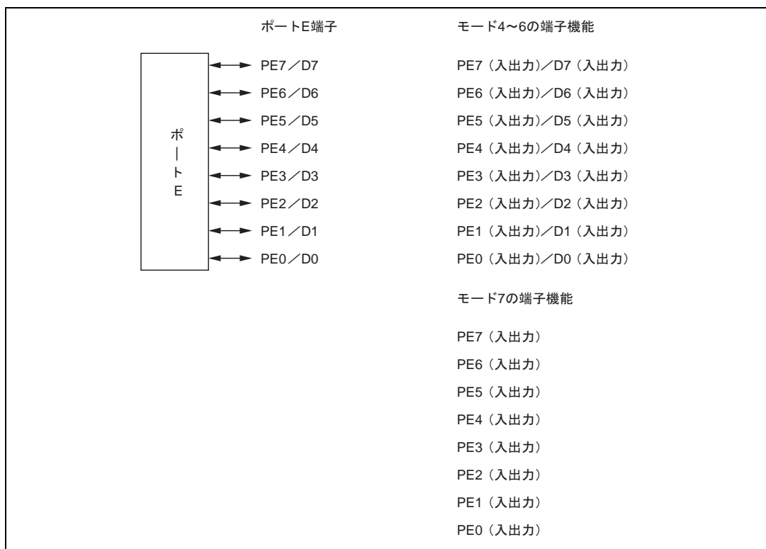
図 9.19 ポート E の端子機能
