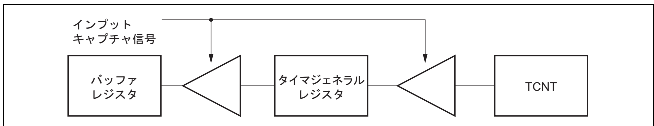
図 13.14 インプットキャプチャバッファ動作
