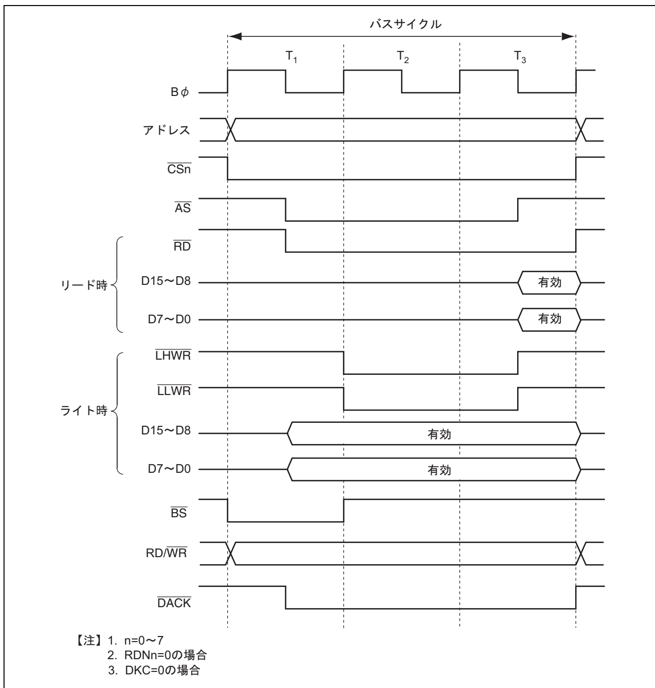
図 9.19 16 ビット 3 ステートアクセス空間のバスタイミング (偶数アドレスワードアクセス)
