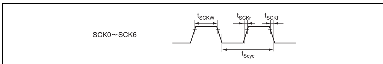
図 27.33 SCK クロック入力タイミング
