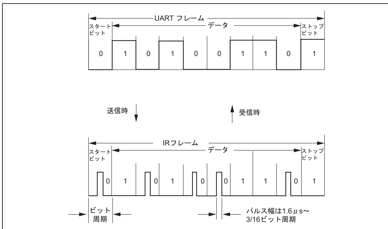
図 17.37 IrDA の送信/受信動作
