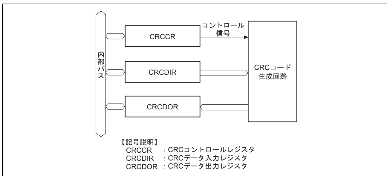
図 17.43 CRC 演算器のブロック図
