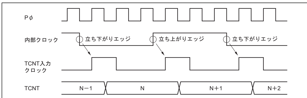
図 13.31 内部クロック動作時のカウントタイミング
