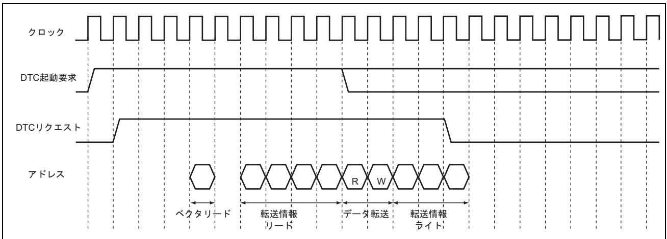
図 11.14 DTC の動作タイミング例 (フルアドレスモード、ノーマル転送モード、リピート転送モード)
