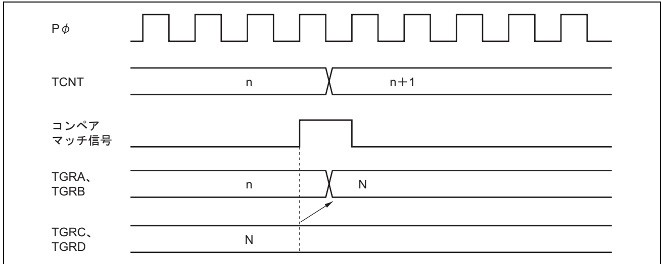
図 13.37 バッファ動作タイミング (コンペアマッチ)
