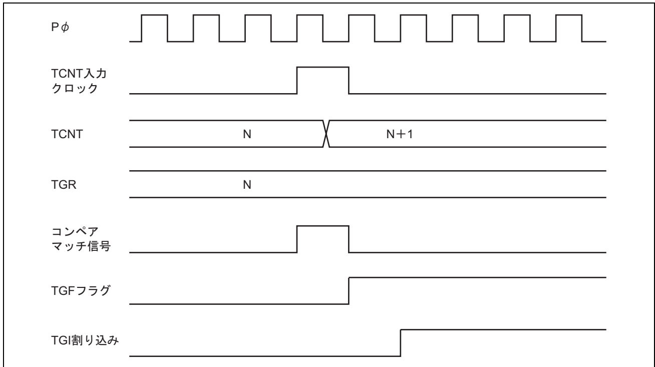
図 13.39 TGI 割り込みタイミング (コンペアマッチ)
