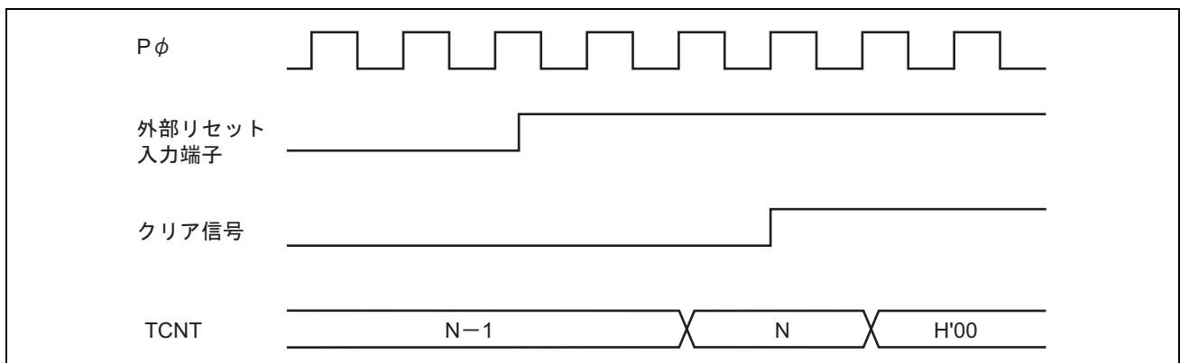
図 15.13 外部リセット入力によるクリアタイミング (ハイレベル)
