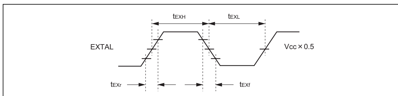
図 24.5 外部クロック入力タイミング
