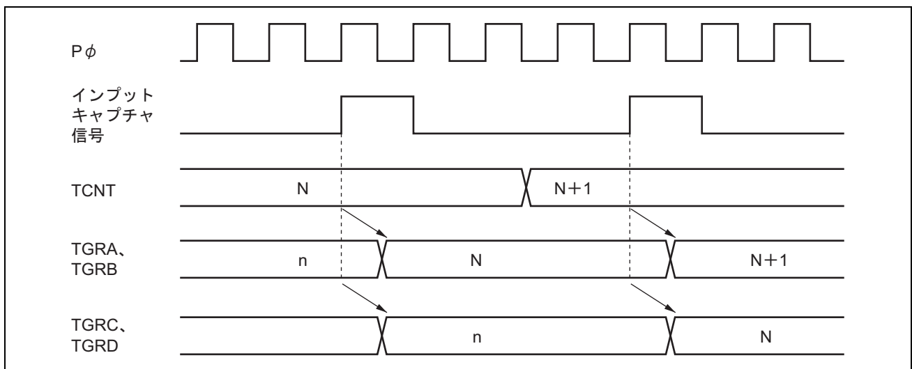
図 13.38 バッファ動作タイミング (入力キャプチャ)
