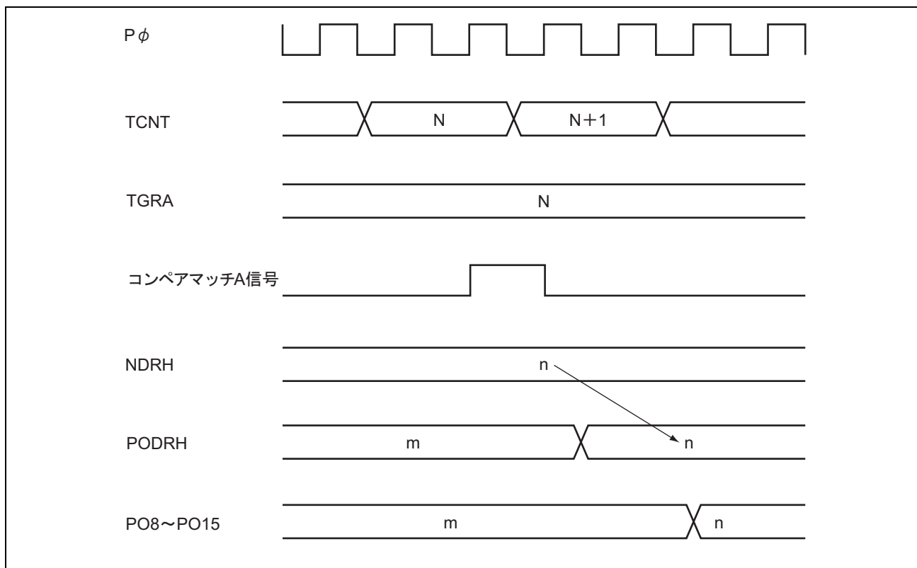
図 14.4 NDR の内容が転送・出力されるタイミング例
