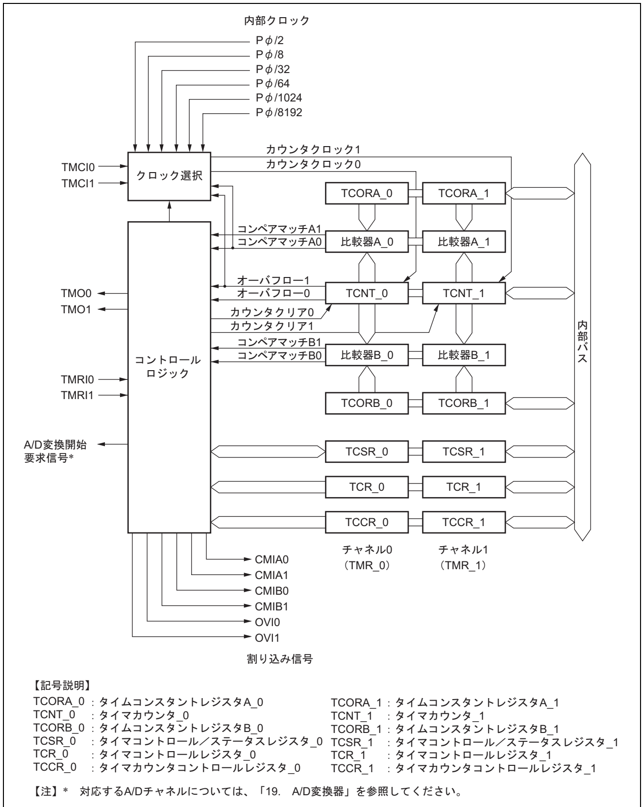
図 15.1 8ビットタイマ (ユニット0) のブロック図
