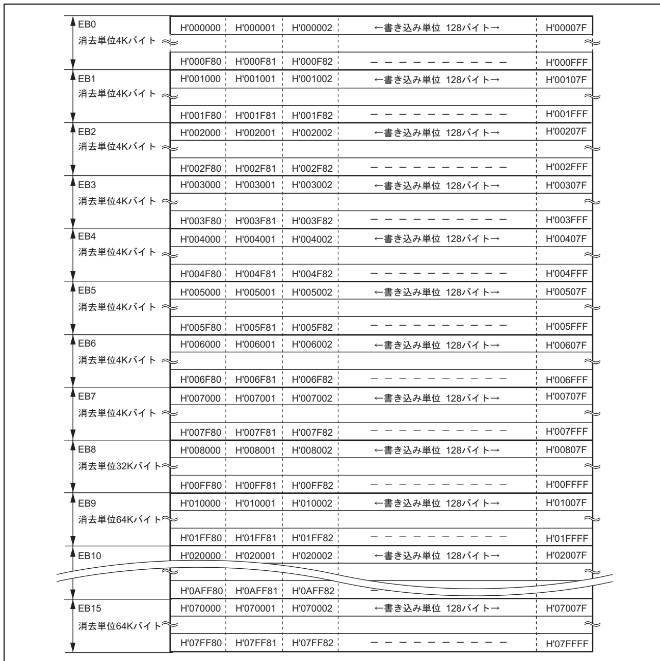
図 22.4 (2) H8SX/1634 のユーザマットのブロック構成
