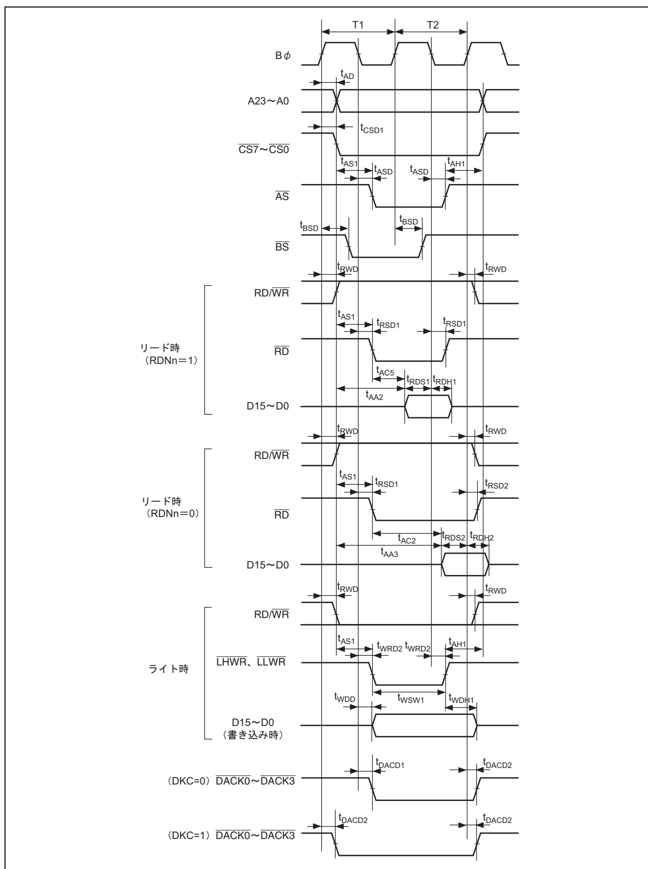
図 27.8 基本バスタイミング/2 ステートアクセス
