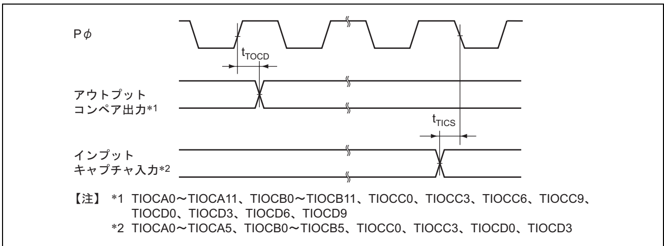
図 27.26 TPU 入出力タイミング
