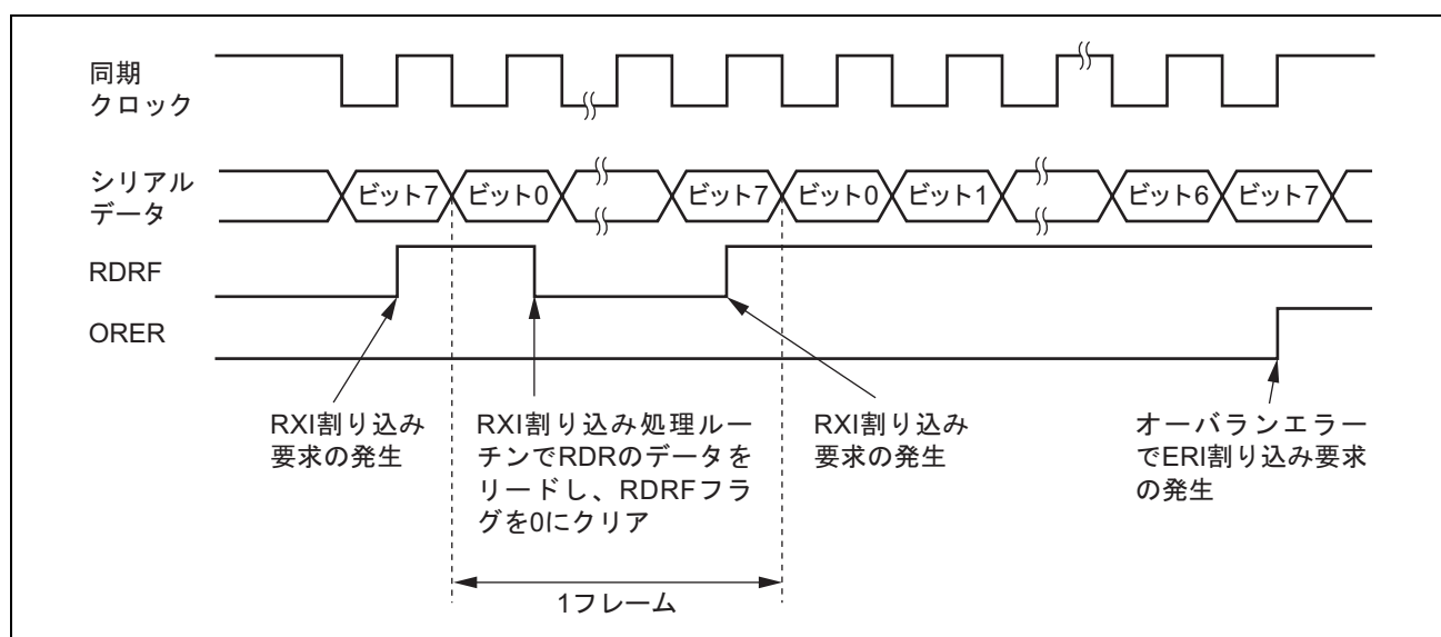
図 17.21 SCI の受信時の動作例
