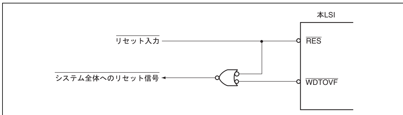
図 16.6 \overline{\text{WDTOVF}} 信号によるシステムのリセット回路例
