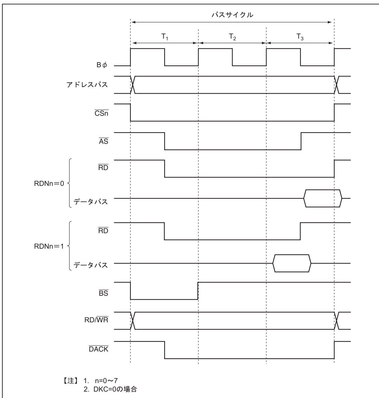
図 9.21 リードストロブタイミング例
