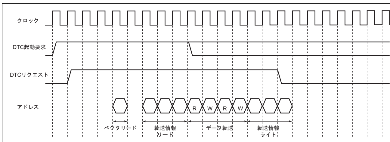
図 11.12 DTC の動作タイミング例 (ショートアドレスモード、ブロック転送モード、ブロックサイズ=2)
