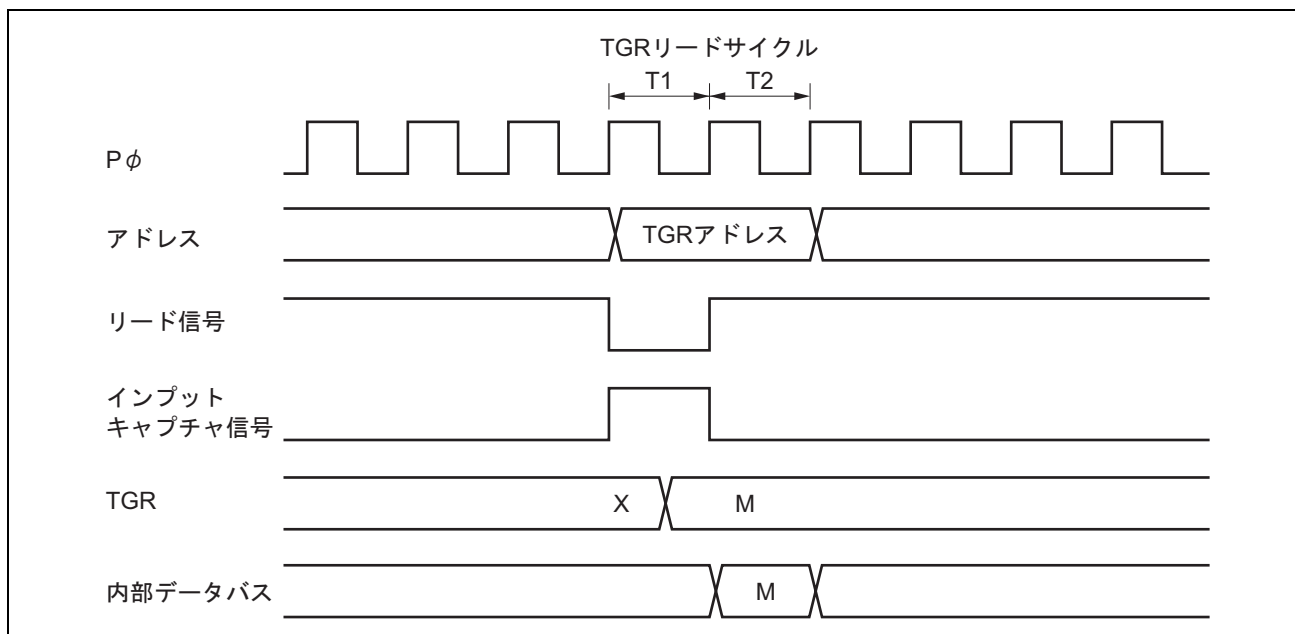
図 13.51 TGRのリードと入力キャプチャの競合
