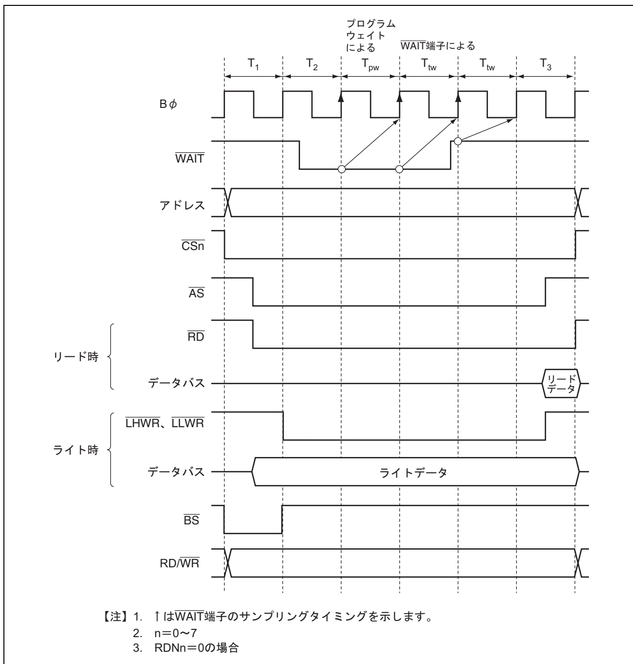
図 9.20 ウェイトステート挿入タイミング例
