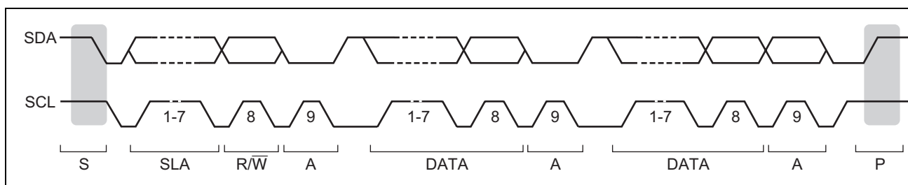
図 18.4 I 2 C バスタイミング
