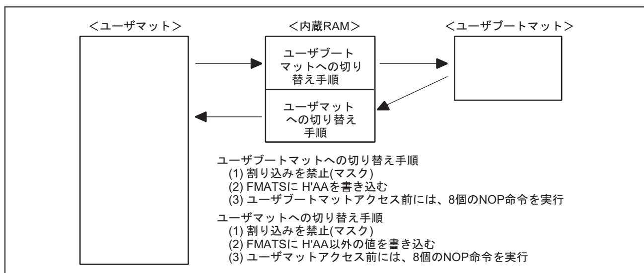
図 22.20 ユーザマット/ユーザブートマットの切り替え
