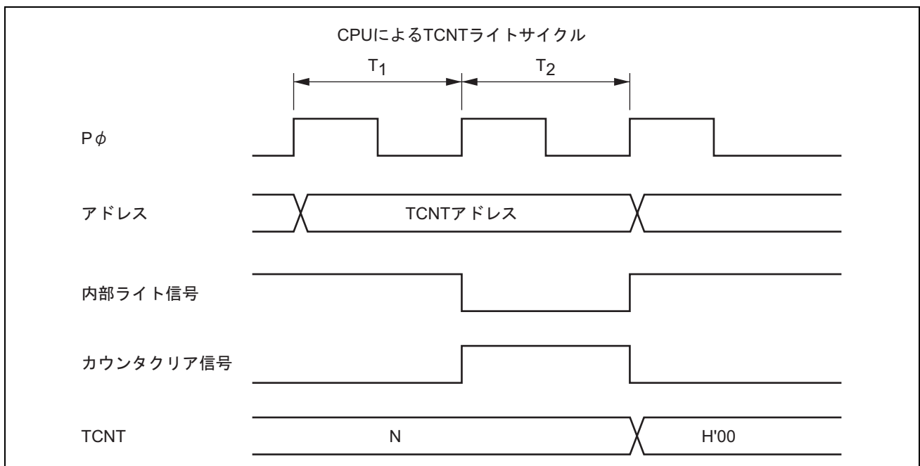
図 15.15 TCNT のライトとクリアの競合
