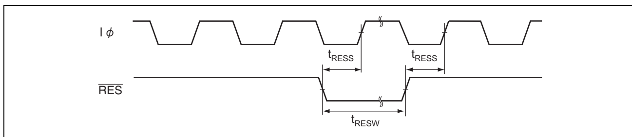
図 27.6 リセット入力タイミング
