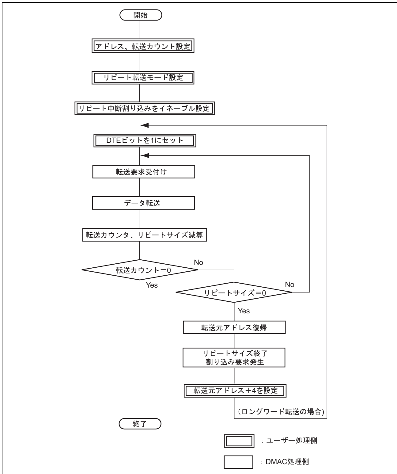
図 10.20 リピート転送モード+オフセット加算によるXY変換のフロー
