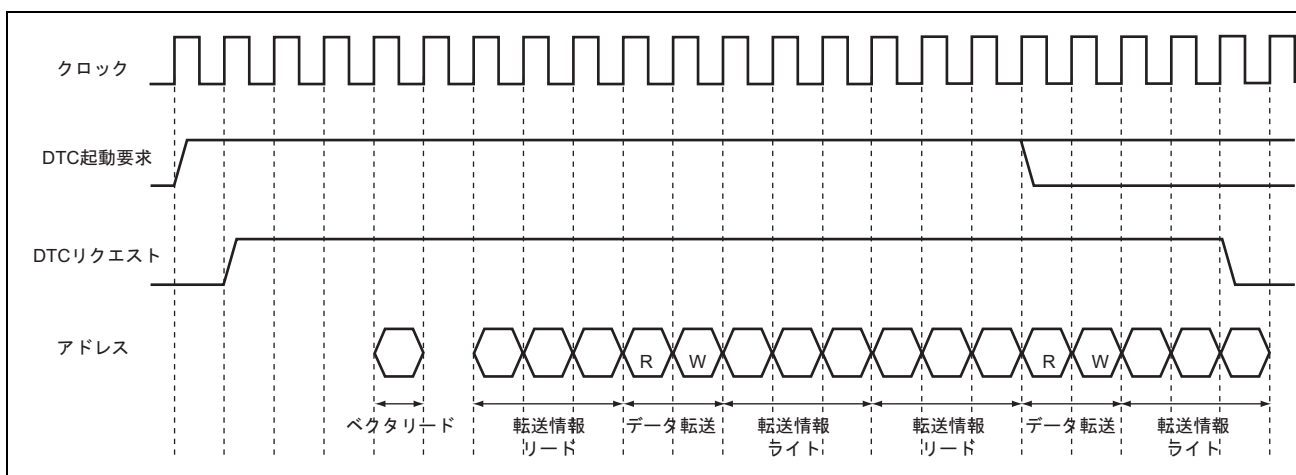
図 11.13 DTC の動作タイミング例 (ショートアドレスモード、チェイン転送)
