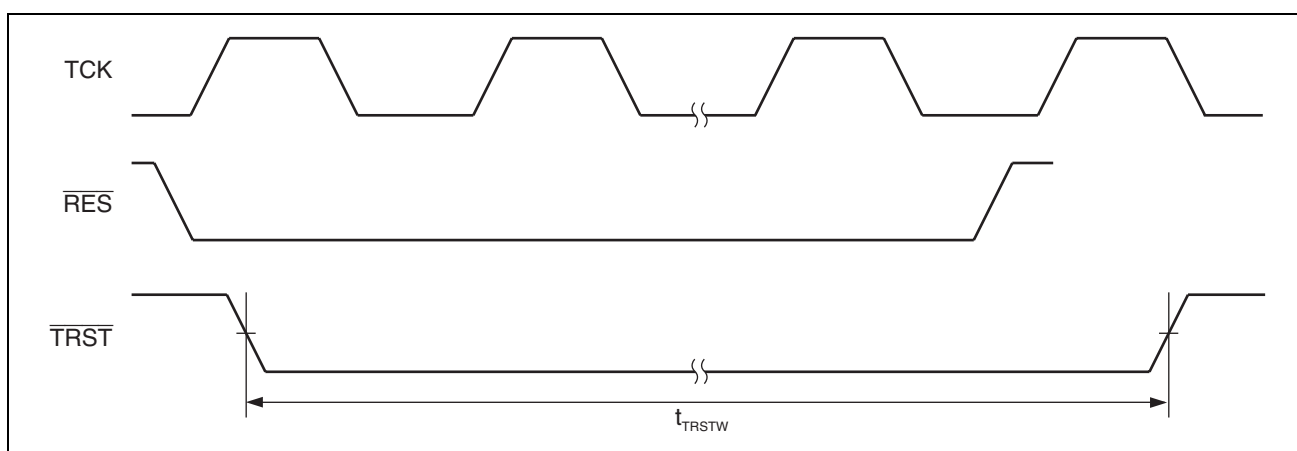
図 27.38 バウンダリスキャン TRST タイミング
