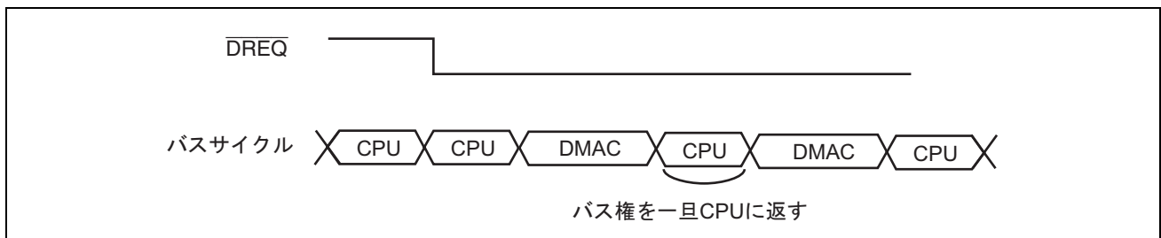
図 10.13 サイクルスチールモードのタイミング例
