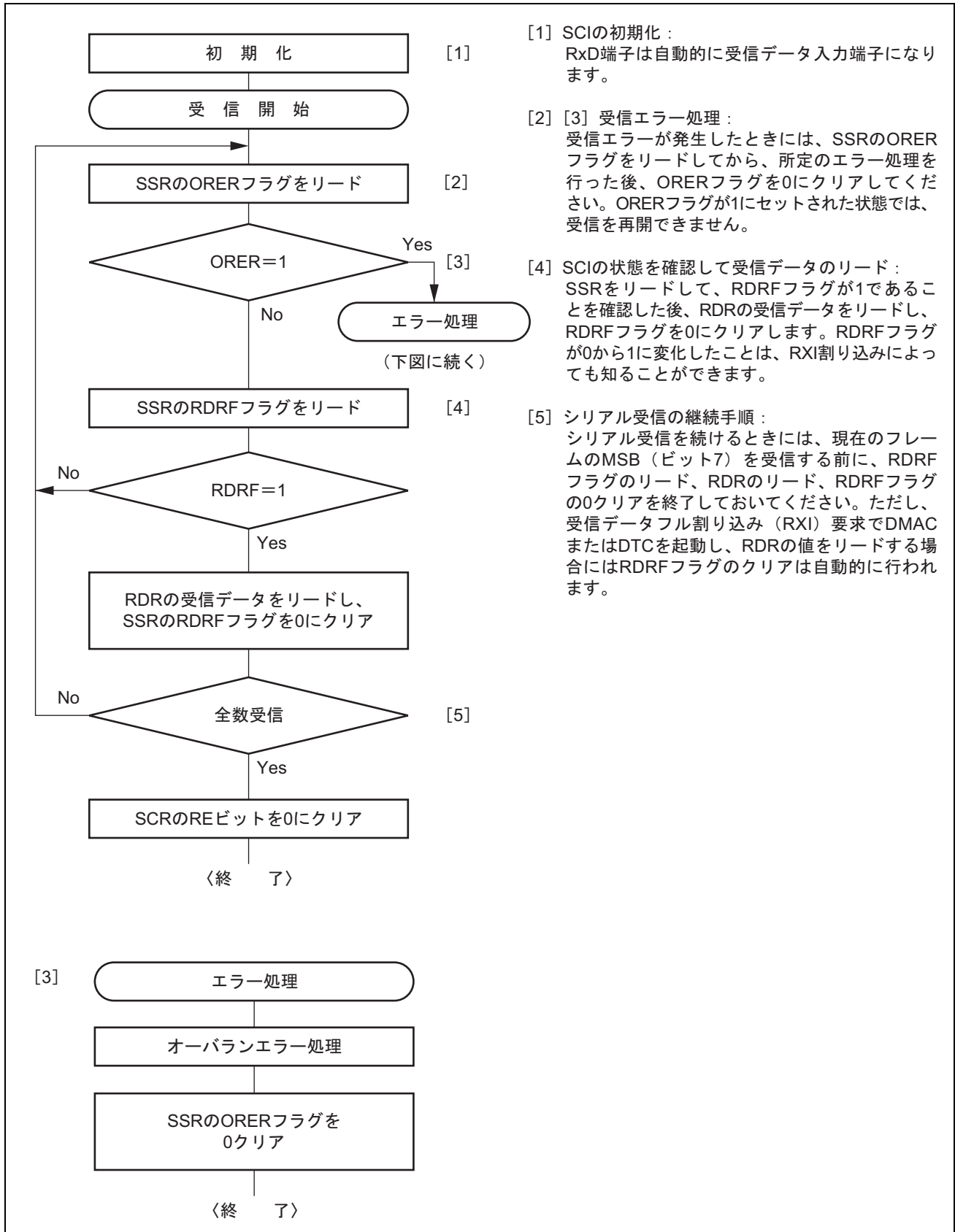
図 17.22 シリアル受信のフローチャートの例
