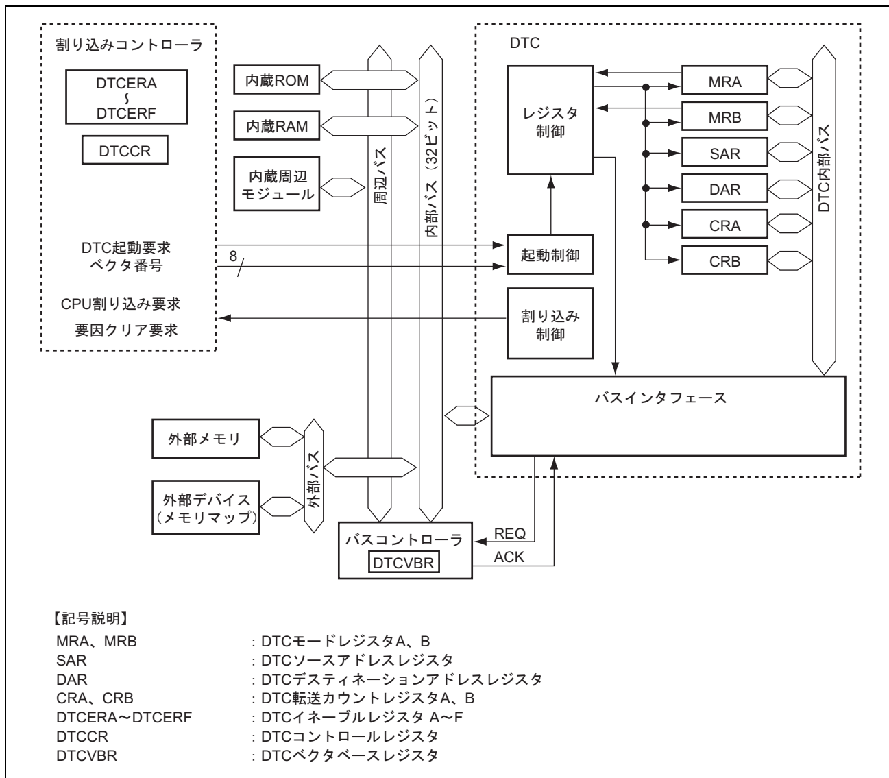
図 11.1 DTC のブロック図
