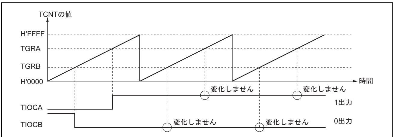
図 13.7 0出力/1出力の動作例
