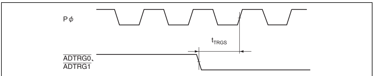
図 27.35 A/D 変換器外部トリガ入力タイミング
