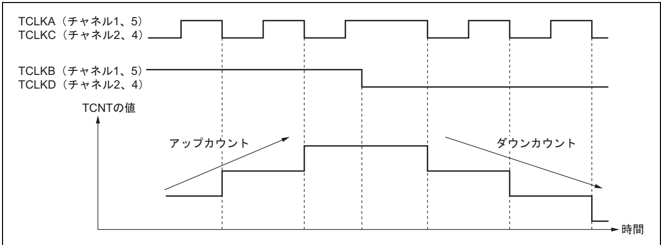
図 13.27 位相計数モード2の動作例
