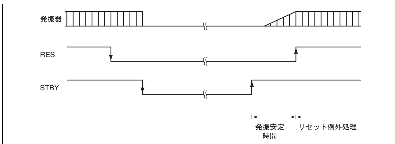
図 25.8 ハードウェアスタンバイモードのタイミング
