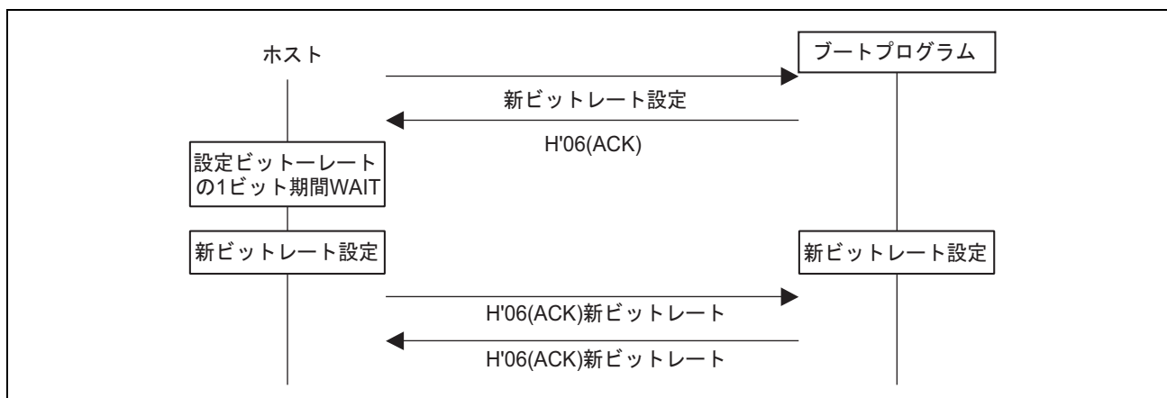
図 22.24 新ビットレート選択のシーケンス
