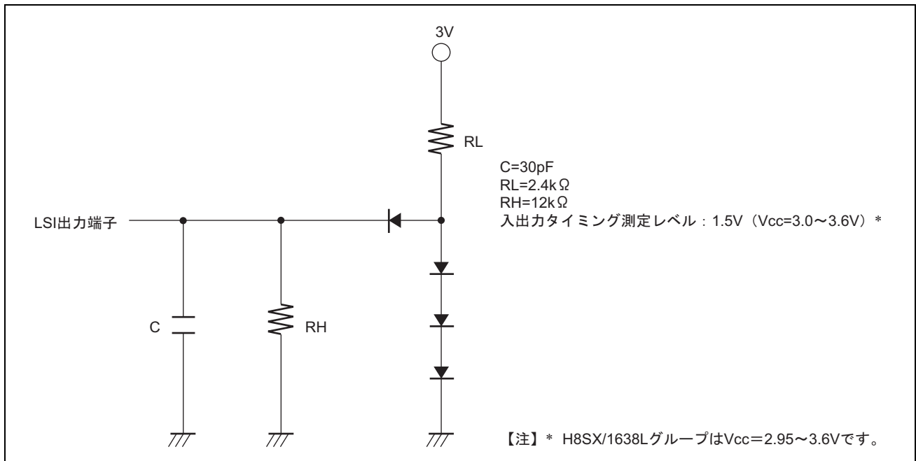
図 27.1 出力負荷回路
