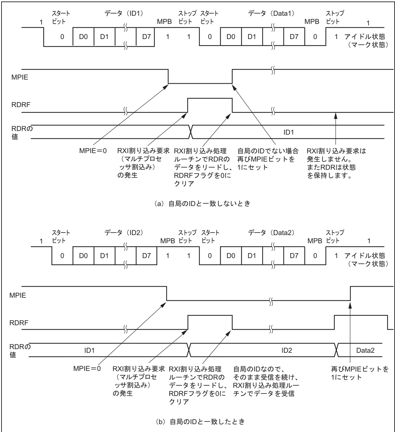
図 17.15 SCI の受信時の動作例 (8 ビットデータ/マルチプロセッサビットあり/1 ストップビットの例)
