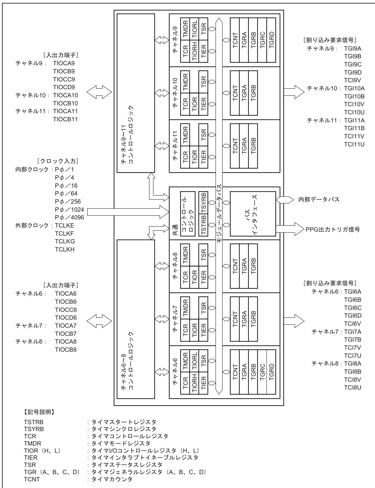
図 13.2 TPU (ユニット1) のブロック図
