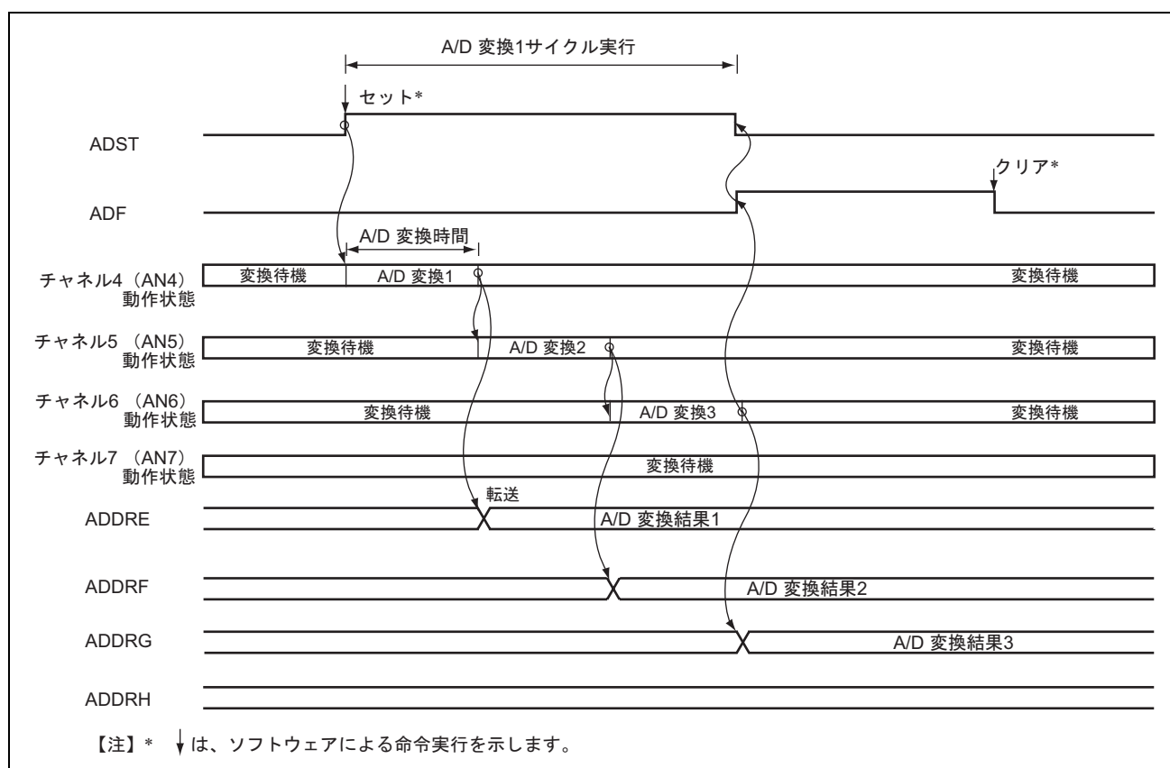
図 19.5 A/D 変換器の動作例（1 サイクルスキャンモード、AN4～AN6 の 3 チャンネル選択時）
