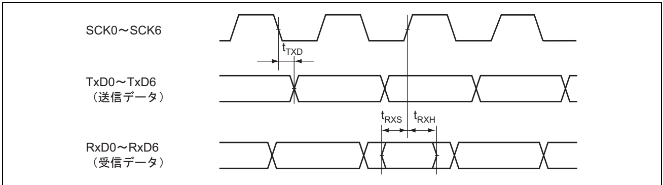
図 27.34 SCI 入出力タイミング/クロック同期式モード
