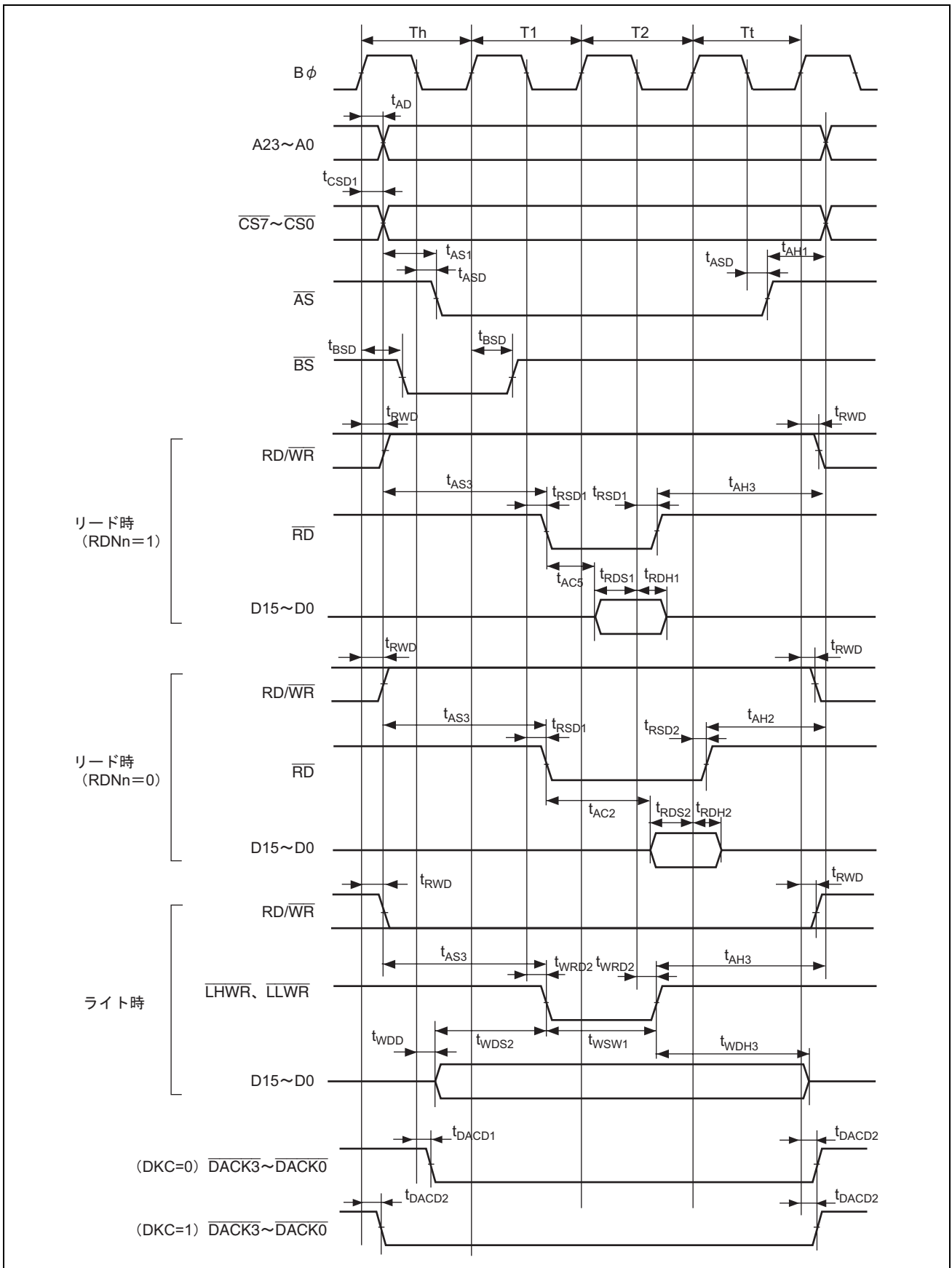
図 27.11 基本バスタイミング/2 ステートアクセス (CS アサート期間延長)
