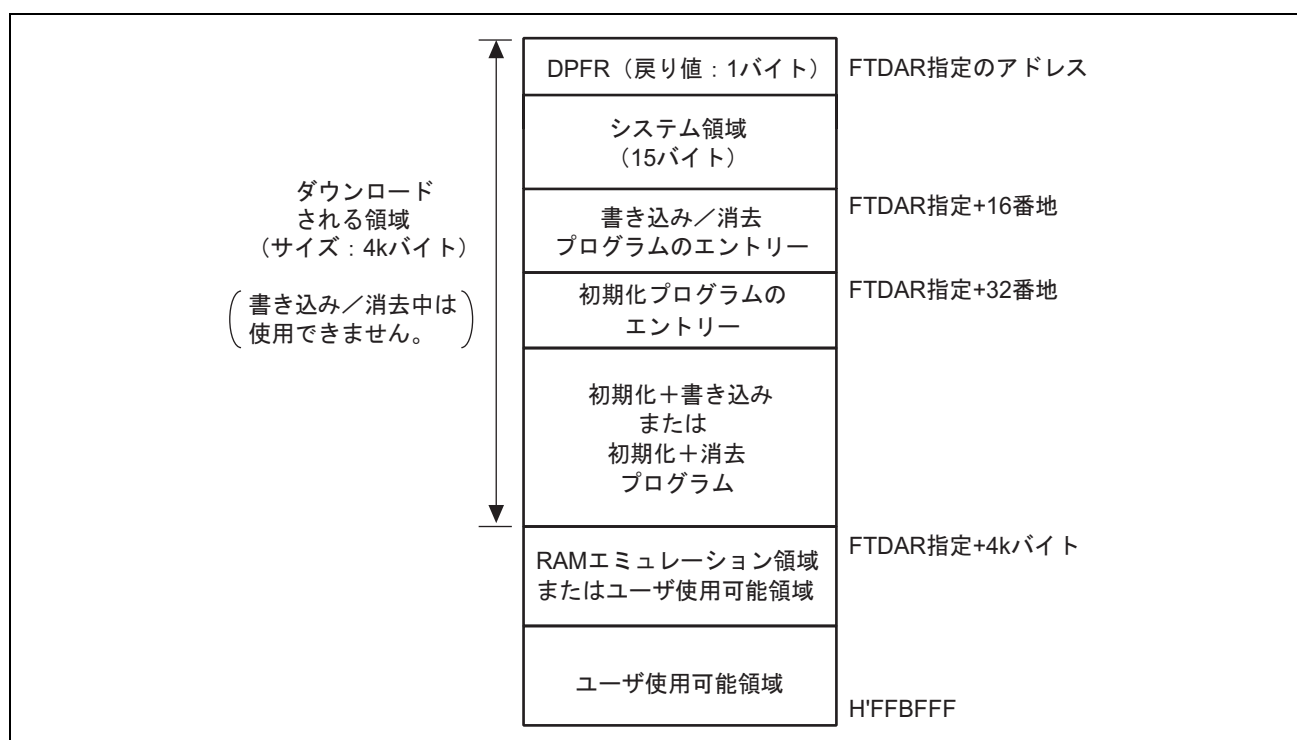
図 22.10 書き込み/消去実行時の RAM マップ
