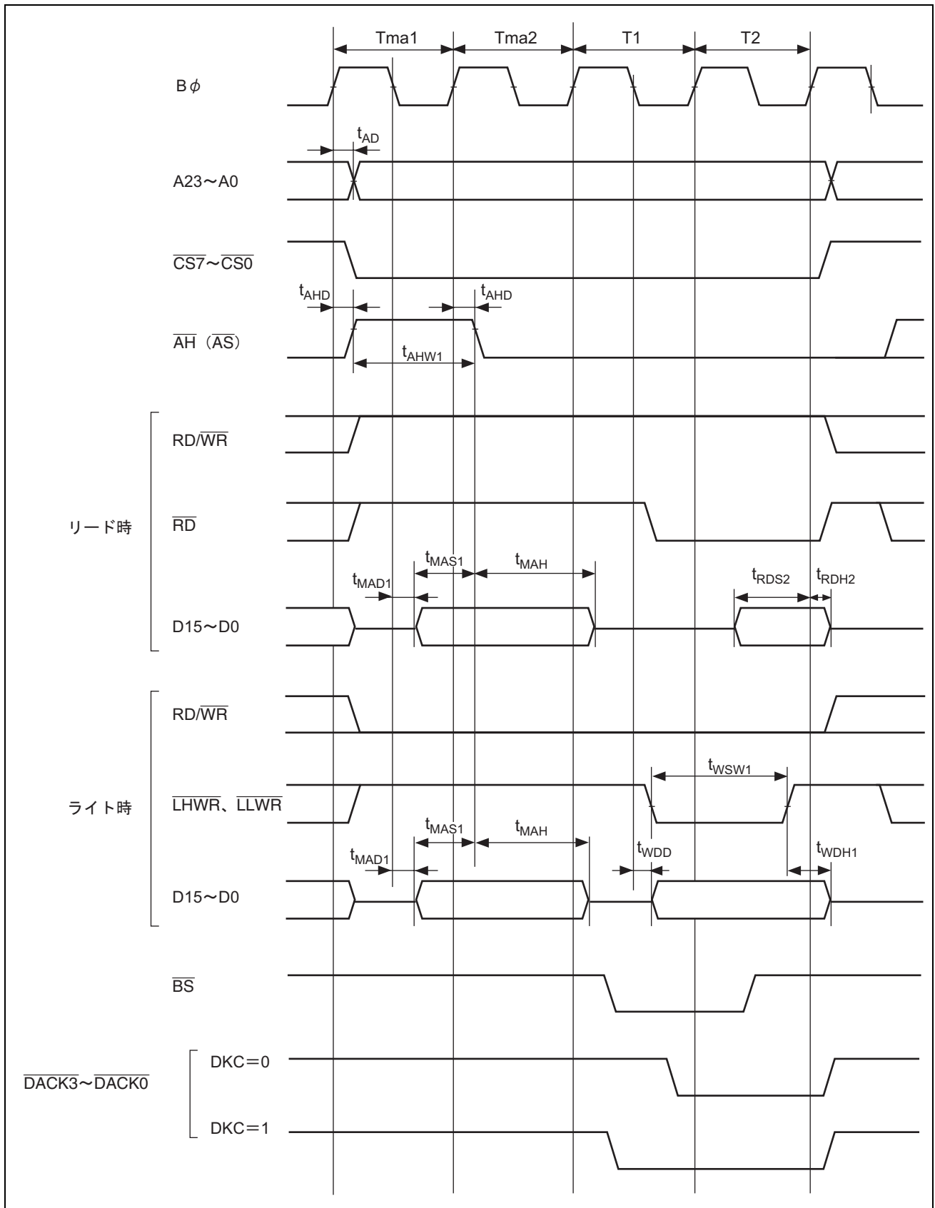
図 27.17 アドレス/データマルチプレクス・アクセスタイミング (ノーウェイト) (-基本・4 ステートアクセス)
