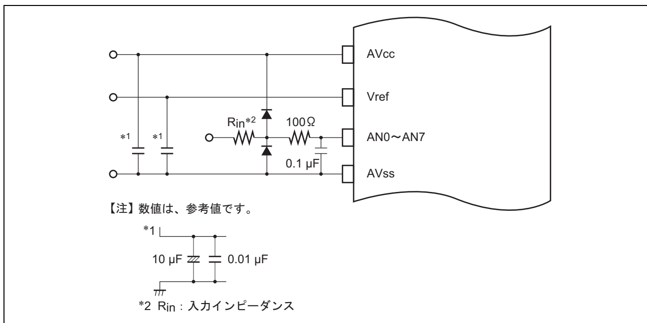
図 19.13 アナログ入力保護回路の例
