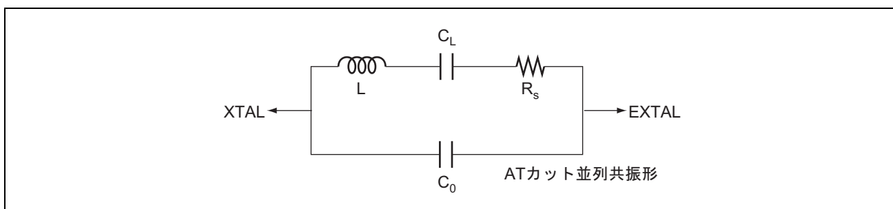
図 24.3 水晶発振子の等価回路
