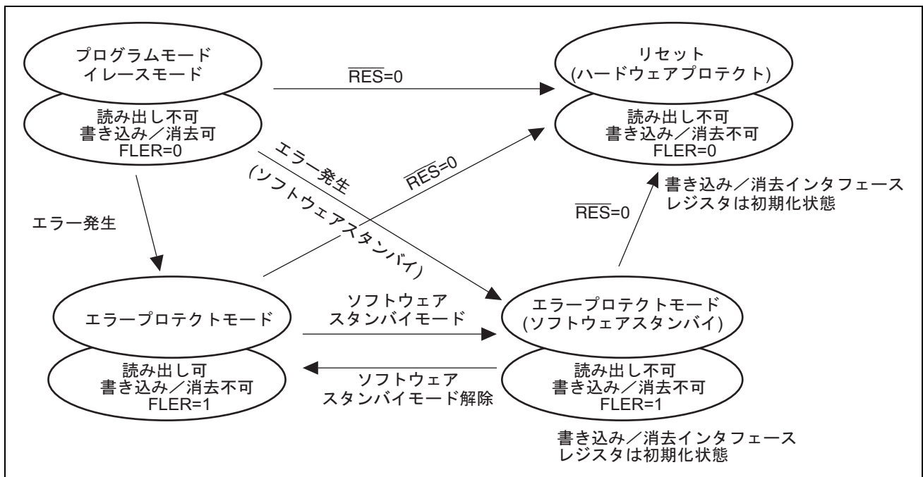
図 22.16 エラープロテクト状態への状態遷移図
