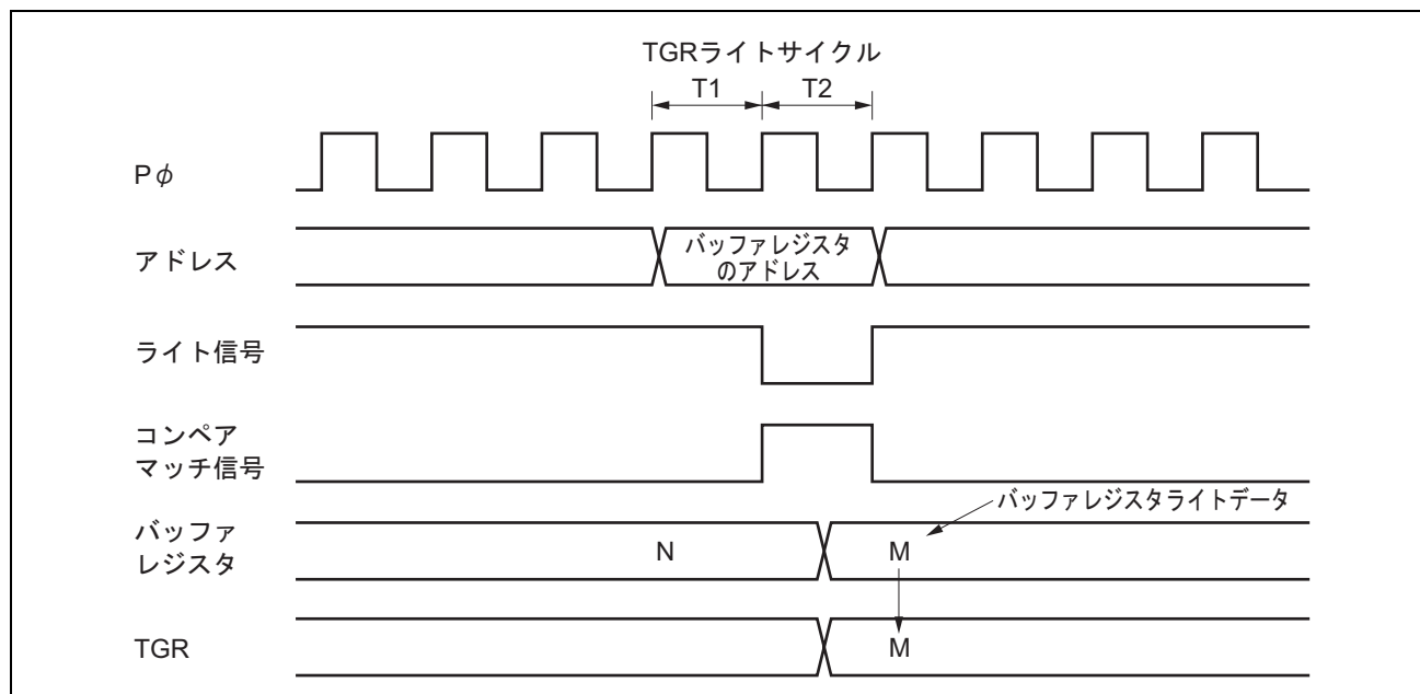
図 13.50 バッファレジスタのライトとコンペアマッチの競合
