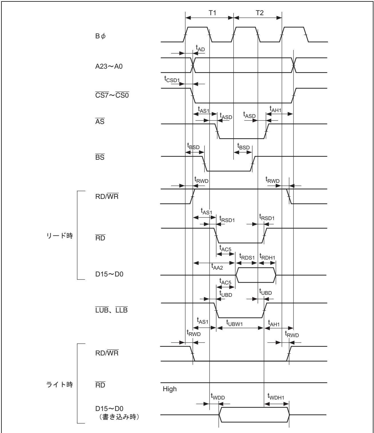
図 27.13 バイト制御 SRAM 2 ステートリード/ライトアクセス
