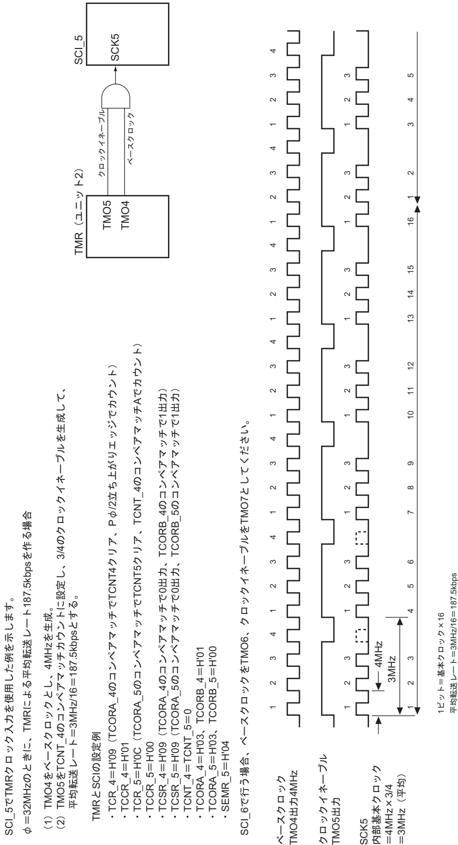
図 17.4 TMR クロック入力時の平均転送レート設定例
