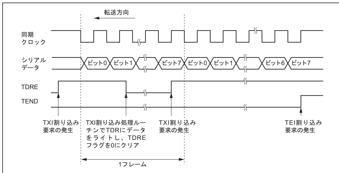
図 17.19 クロック同期式モードの送信時の動作例
