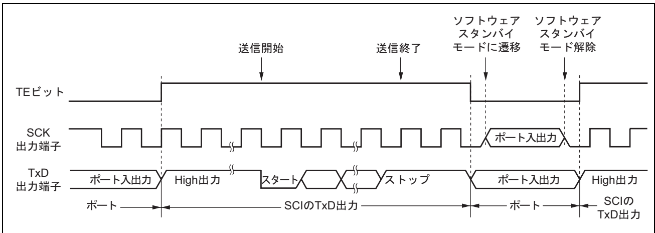
図 17.40 ソフトウェアスタンバイモード遷移時のポートの端子状態 (内部クロック、調歩同期送信)
