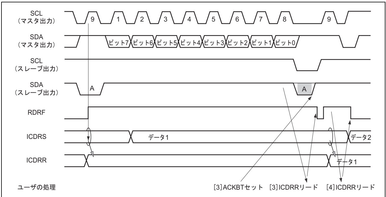
図 18.12 スレーブ受信モード動作タイミング 2
