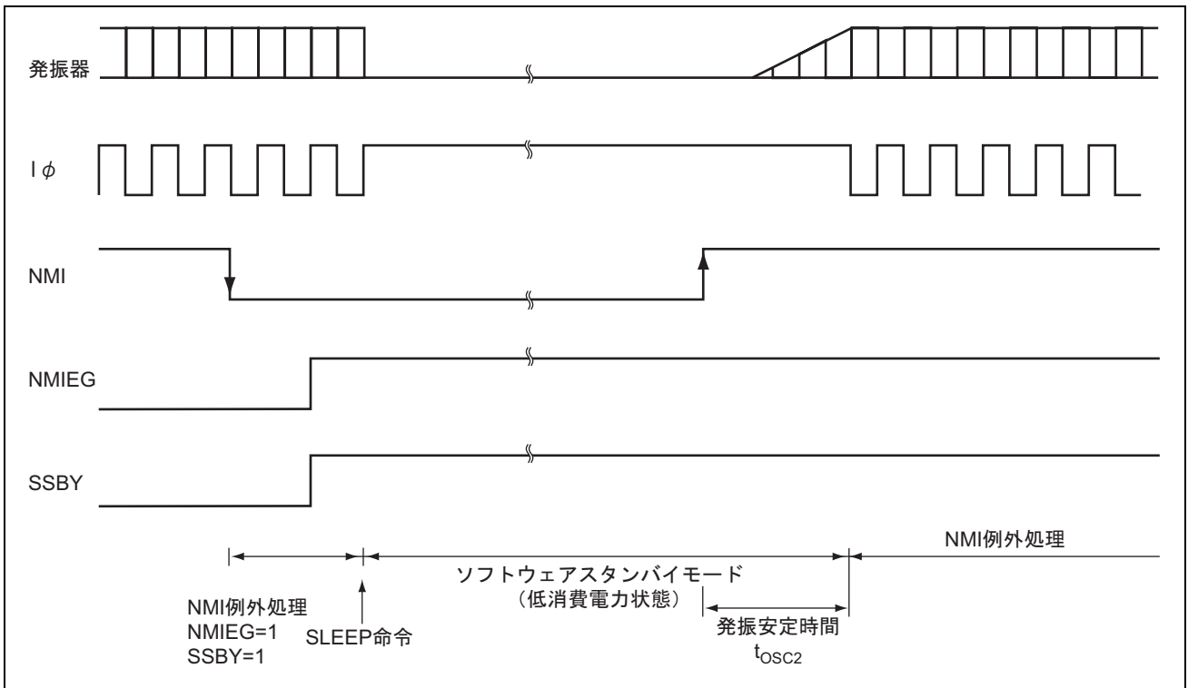
図 27.3 ソフトウェアスタンバイ発振安定時間タイミング
