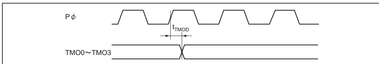
図 27.29 8ビットタイマ出力タイミング
