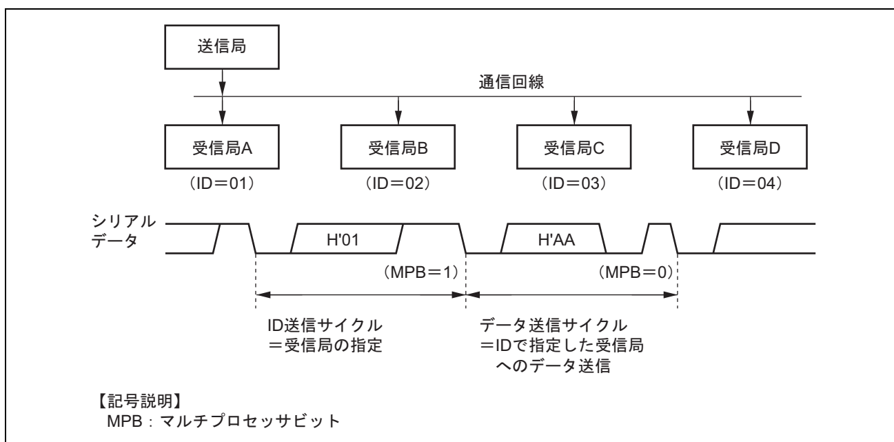
図 17.13 マルチプロセッサフォーマットを使用した通信例 (受信局 A へのデータ H'AA の送信の例)
