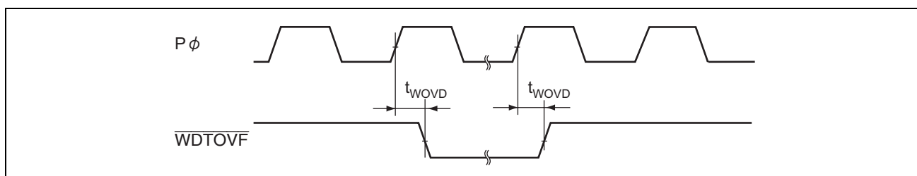
図 27.32 WDT 出力タイミング
