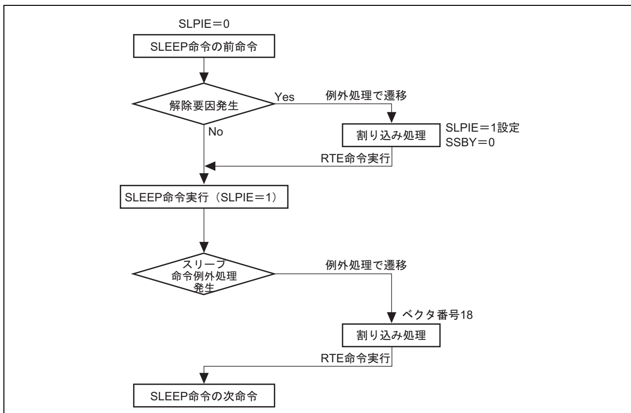
図 25.12 SLEEP 命令実行直前に解除要因割り込みが発生した場合(スリープ命令例外処理が発生する場合)
