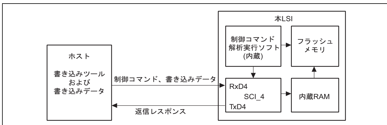
図 22.6 ブートモードのシステム構成図
