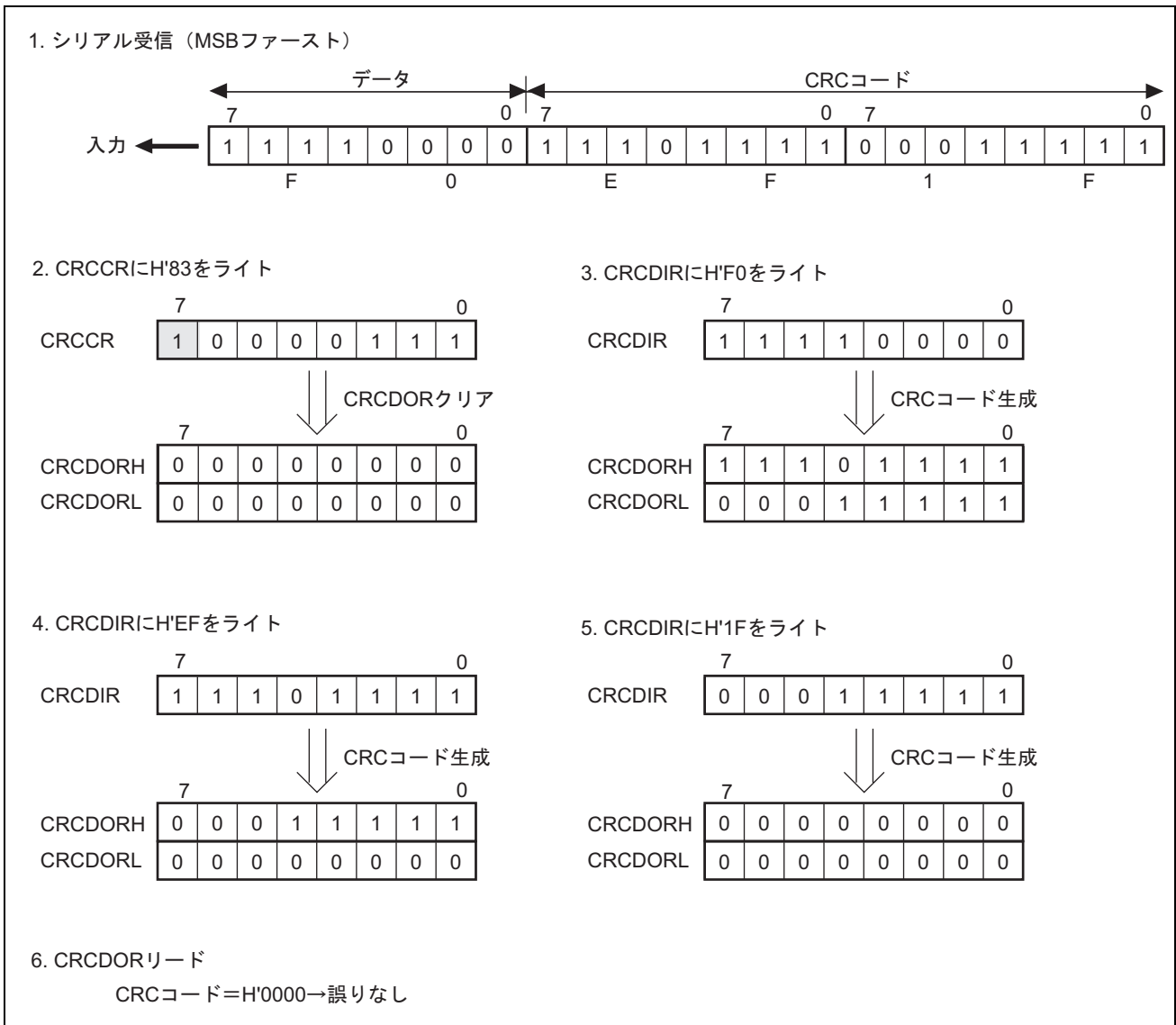
図 17.47 MSB ファーストでのデータ受信
