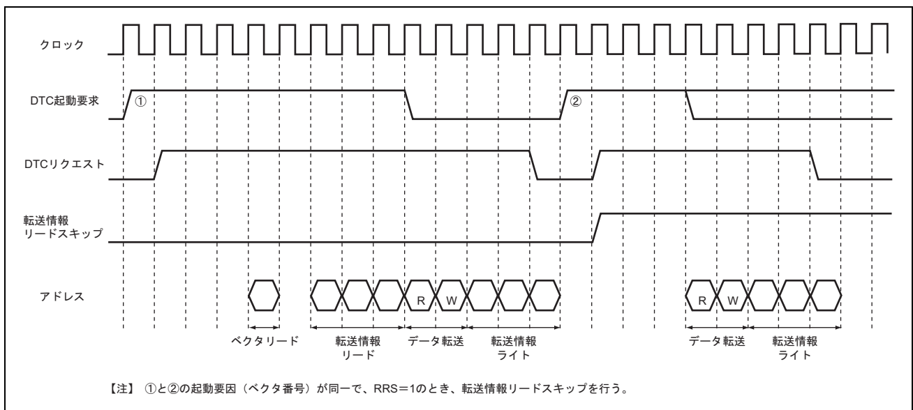
図 11.6 転送情報リードスキップのタイミングチャート
