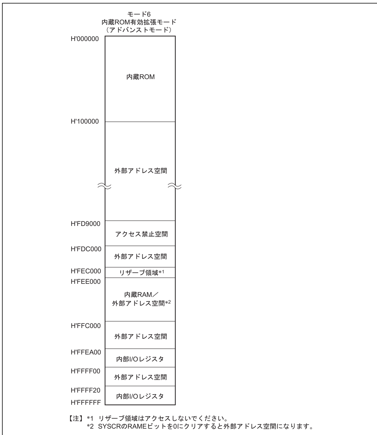
図 3.1 H8SX/1638、1638L の各動作モードのアドレスマップ (2)
