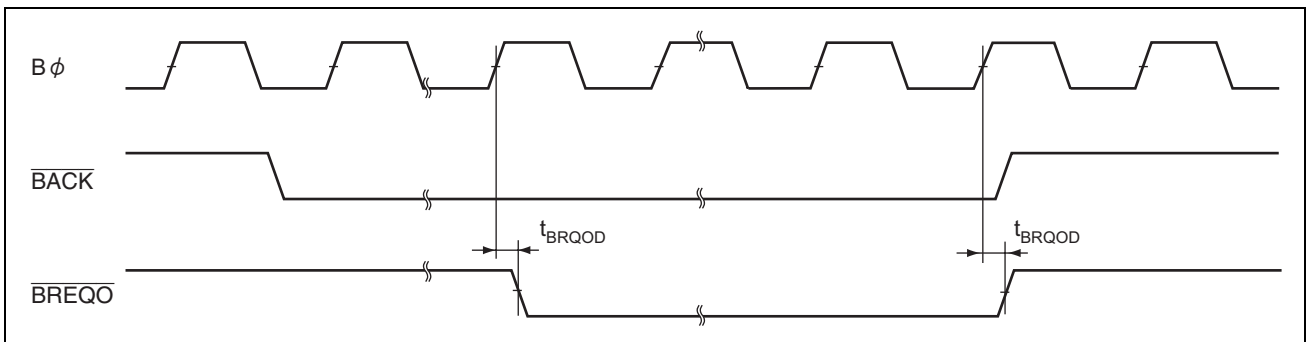
図 27.20 外部バス権要求出力タイミング
