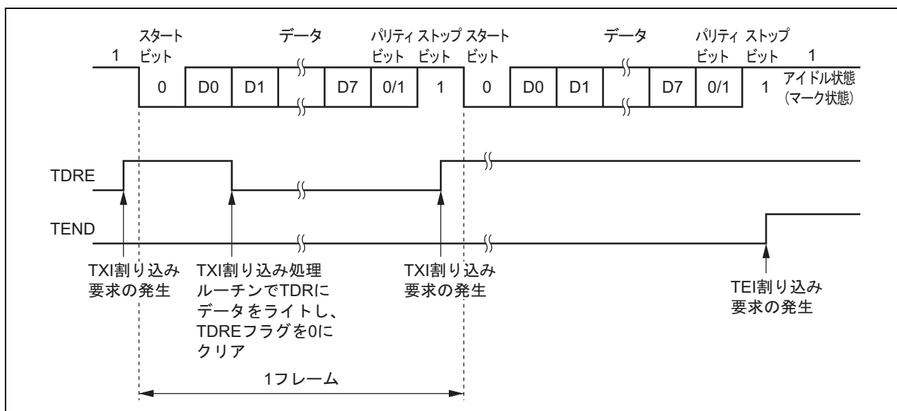
図 17.9 調歩同期式モードの送信時の動作例 (8 ビットデータ/パリティあり/1 ストップビットの例)
