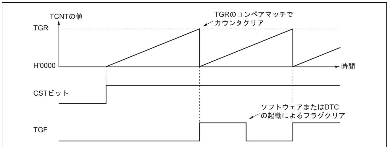
図 13.5 周期カウンタの動作
