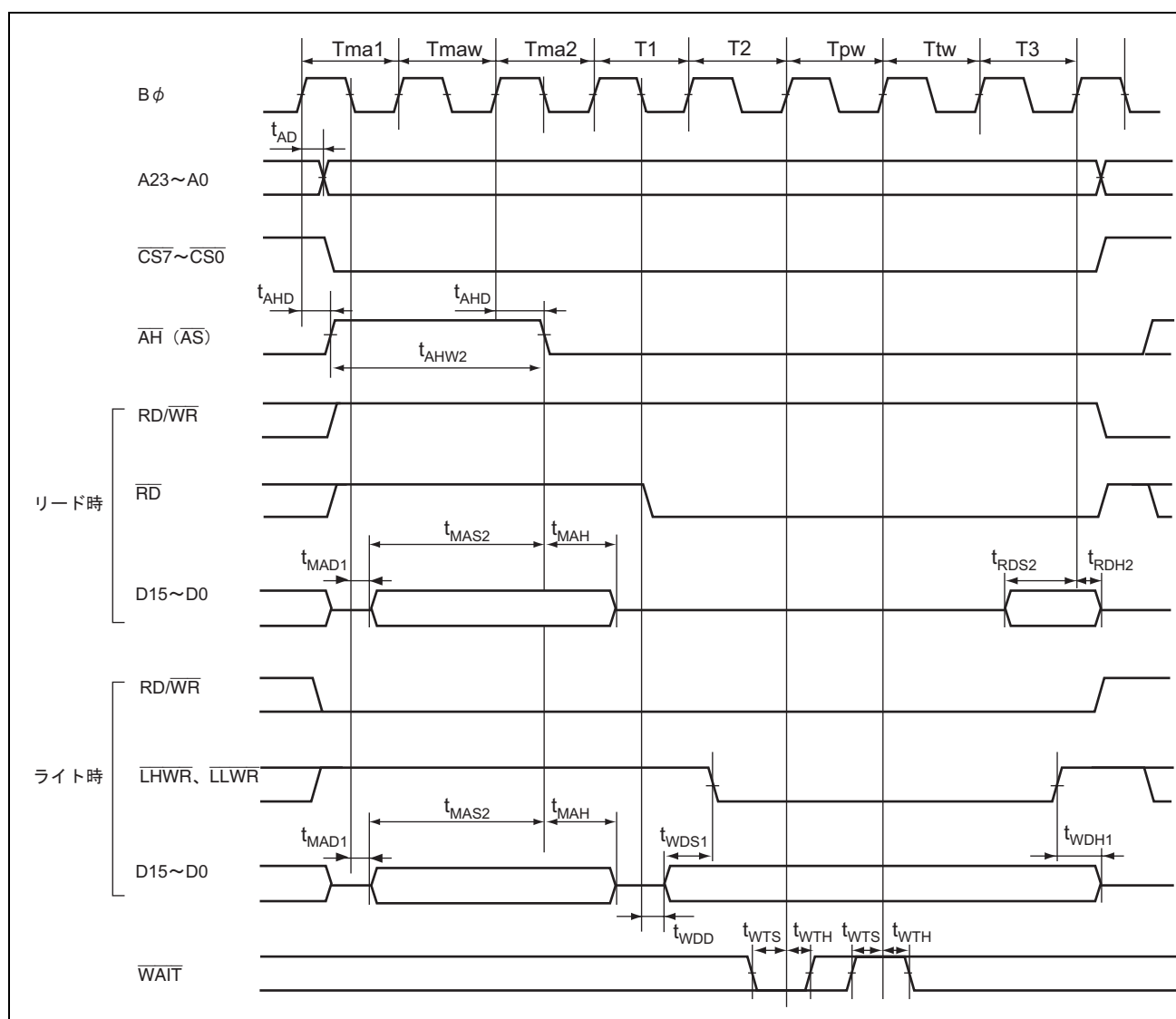
図 27.18 アドレス/データマルチプレクス・アクセスタイミング (ウェイト制御) (-アドレスサイクルプログラムウェイト×1 +データサイクルプログラムウェイト×1+データサイクル端子ウェイト×1の場合)
