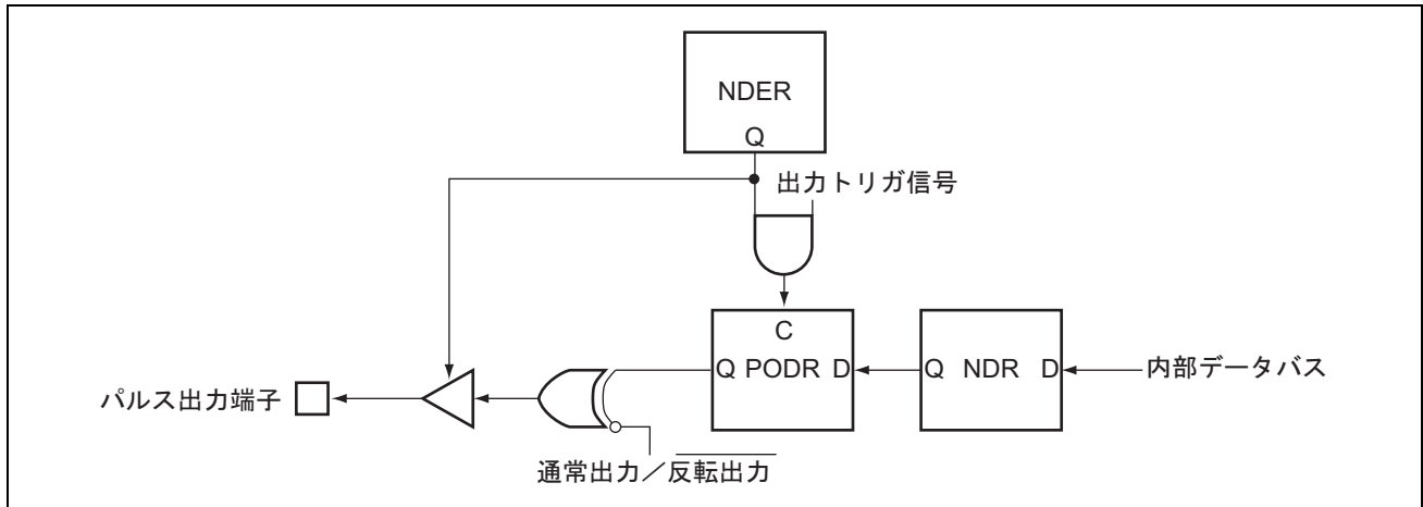
図 14.3 PPG 概要図
