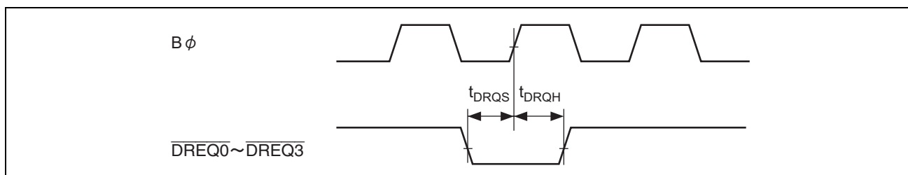
図 27.21 DMAC、 \overline{\text{DREQ}} 入力タイミング
