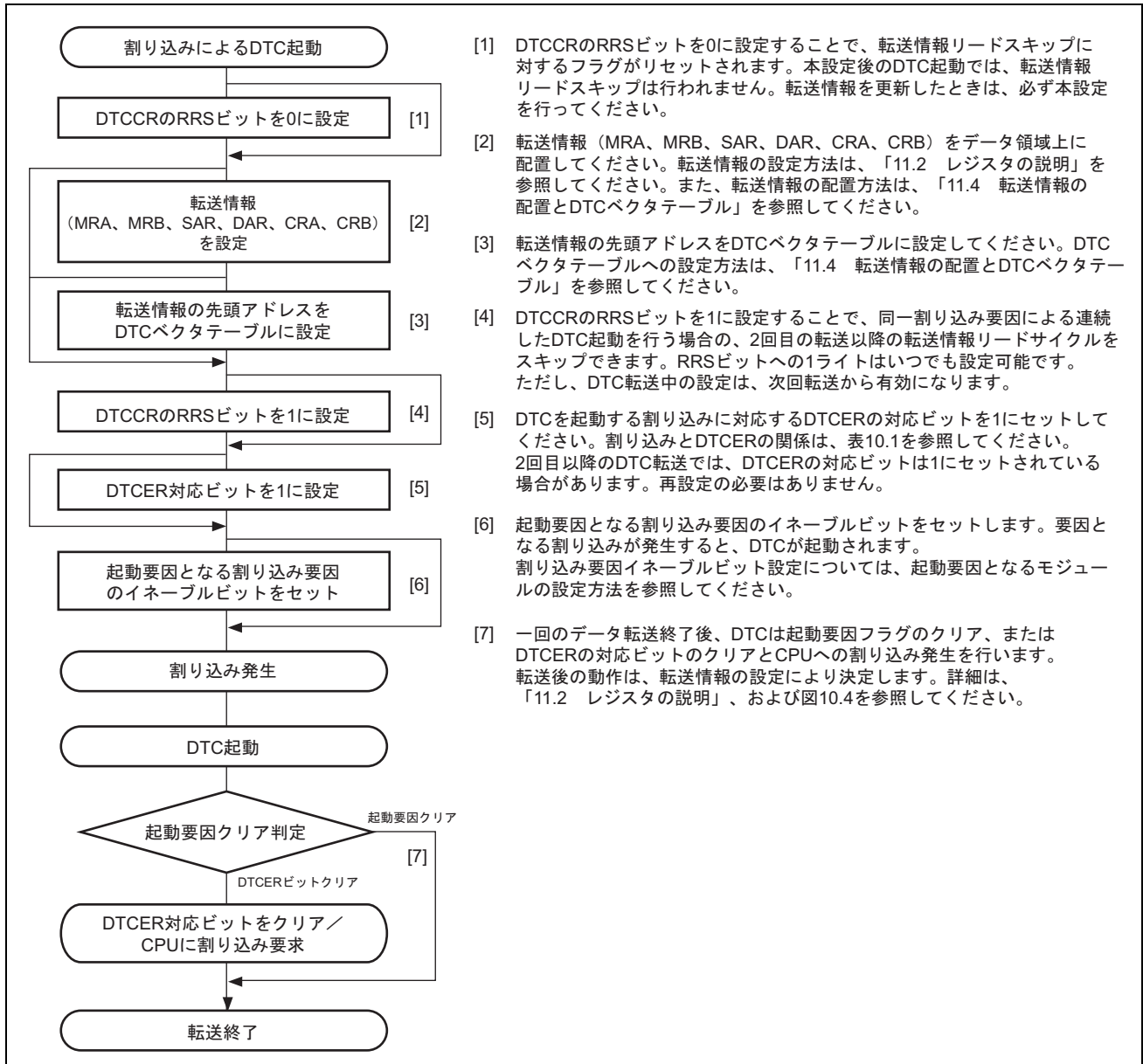
図 11.15 割り込みによる DTC 起動方法
