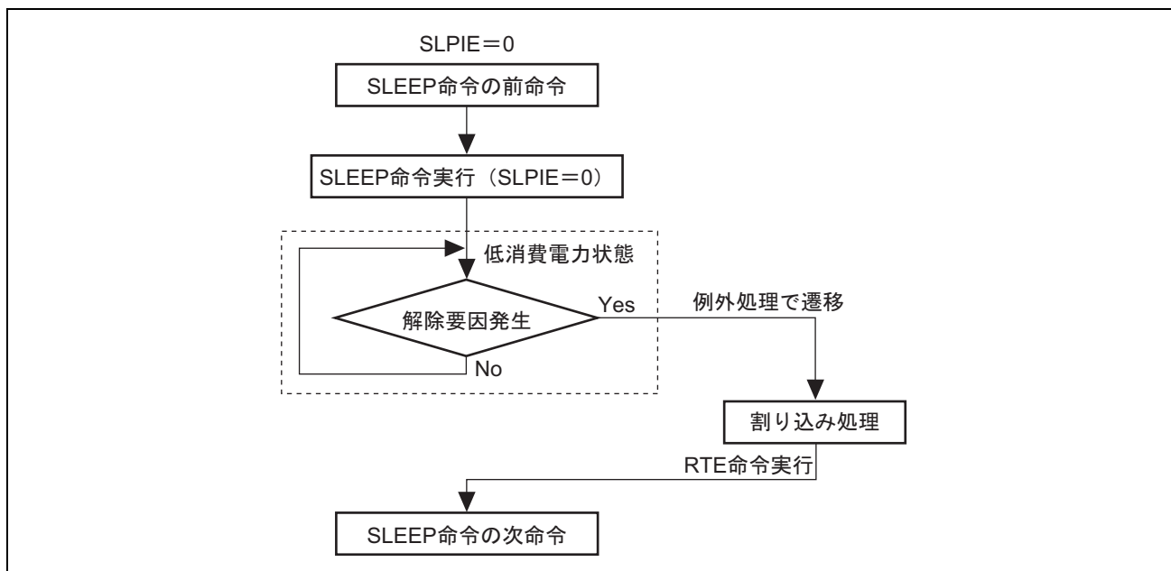
図 25.10 SLEEP 命令実行後に解除要因割り込みが発生した場合
