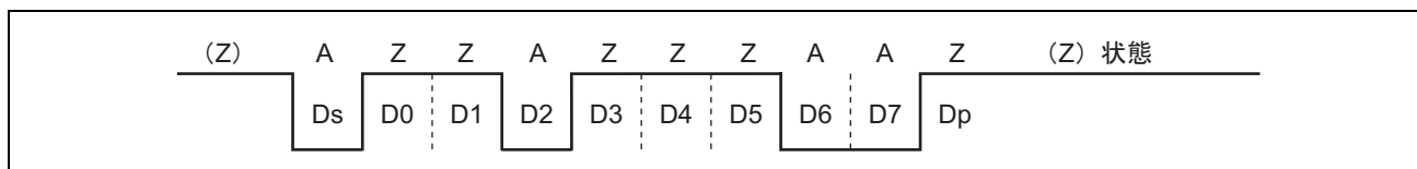
図 17.26 ダイレクトコンベンション (SDIR=SINV=O/E=0)
