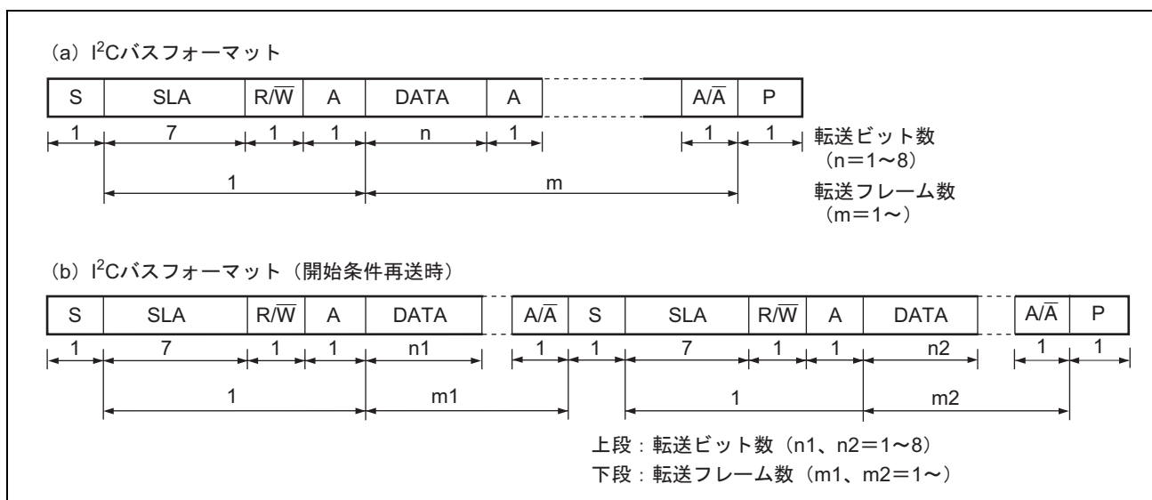
図 18.3 I 2 C バスフォーマット
