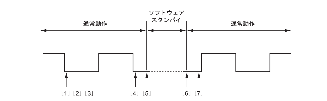
図 17.35 クロック停止・再起動手順
