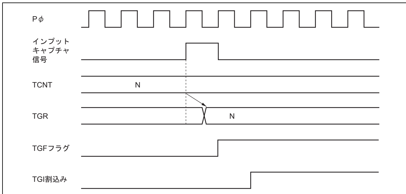
図 13.40 TGI 割り込みタイミング (インพุットキャプチャ)
