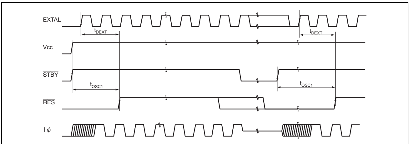
図 27.4 発振安定時間タイミング
