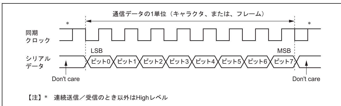
図 17.17 クロック同期式通信のデータフォーマット (LSB ファーストの場合)
