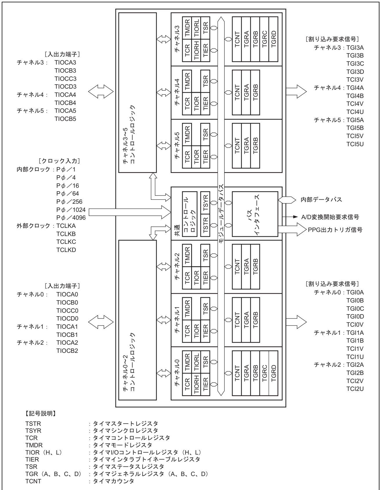
図 13.1 TPU (ユニット0) のブロック図
