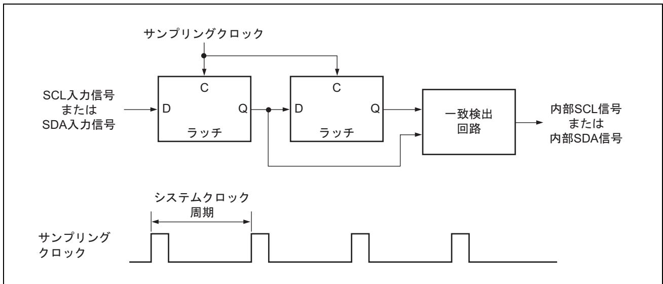
図 18.13 ノイズ除去回路のブロック図
