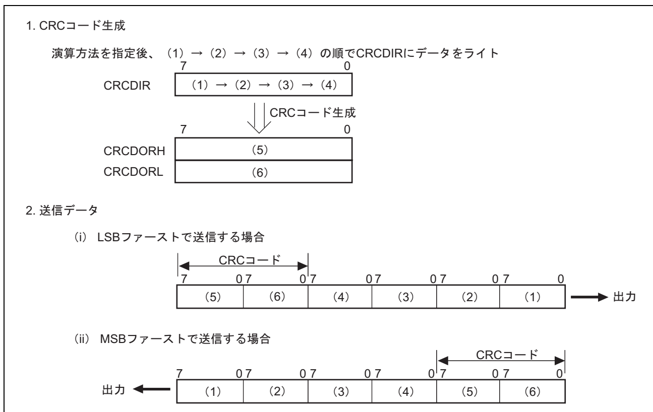
図 17.48 LSB ファーストと MSB ファーストの送信データ
