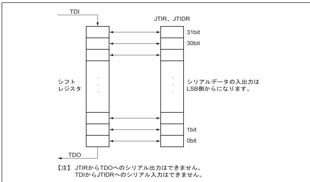
図 23.3 シリアルデータ入出力
