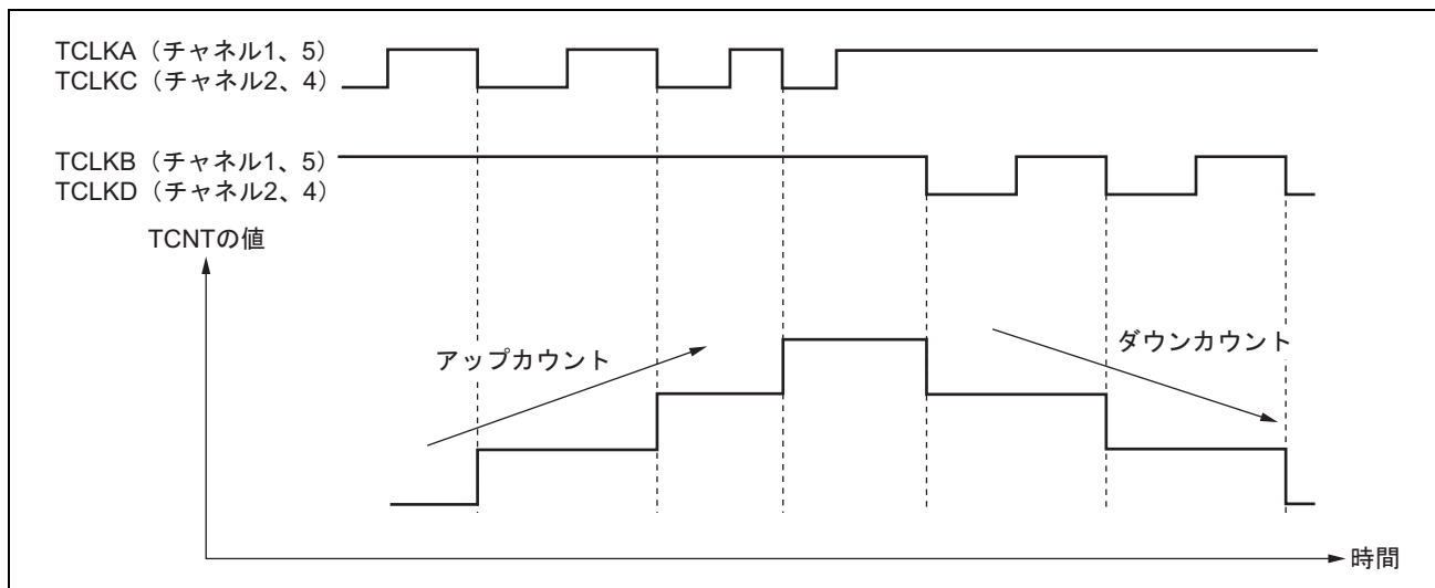
図 13.28 位相計数モード 3 の動作例
