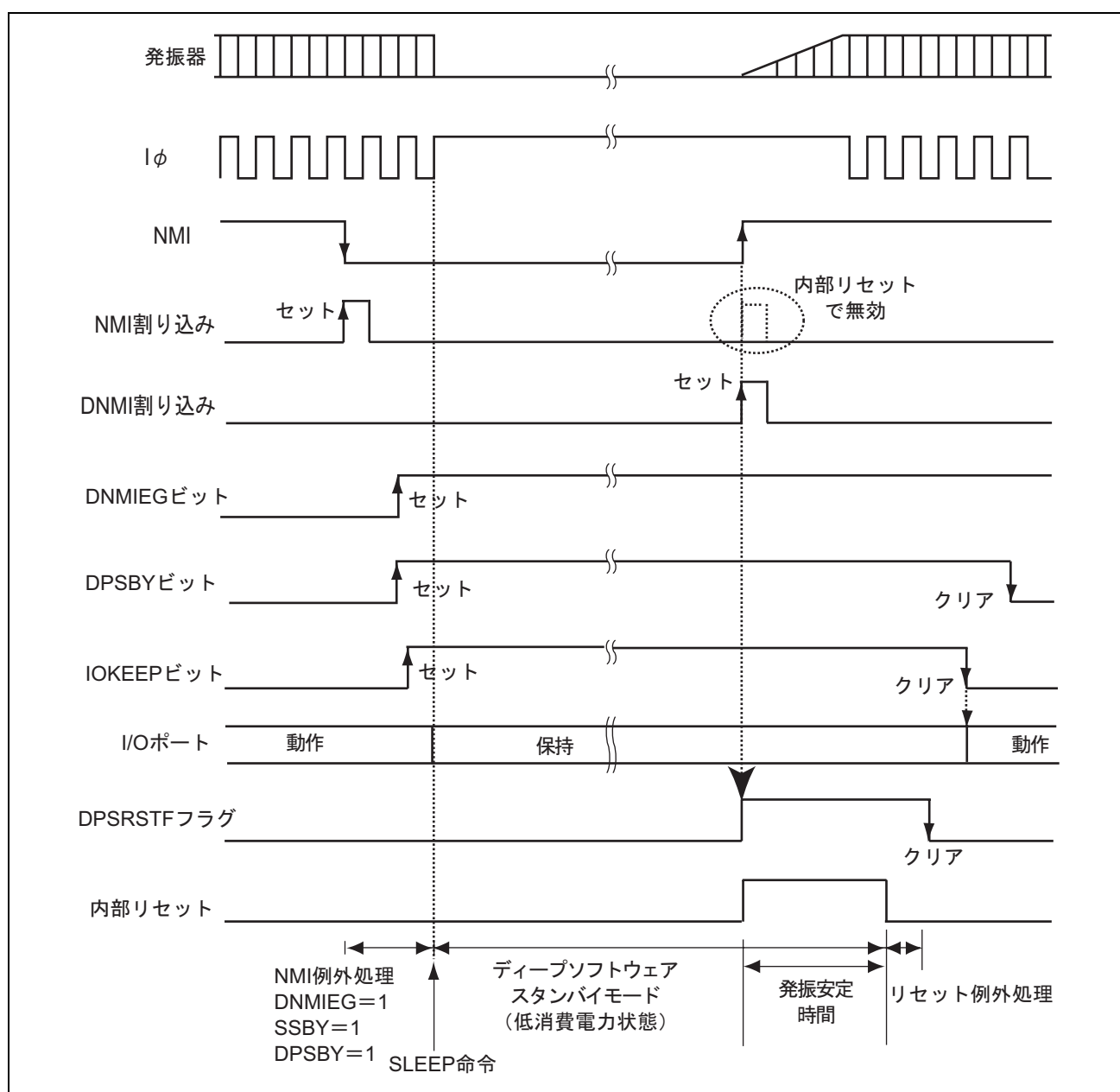
図 25.4 ディープソフトウェアスタンバイモードの応用例 (IOKEEP ビットが 1 のとき)
