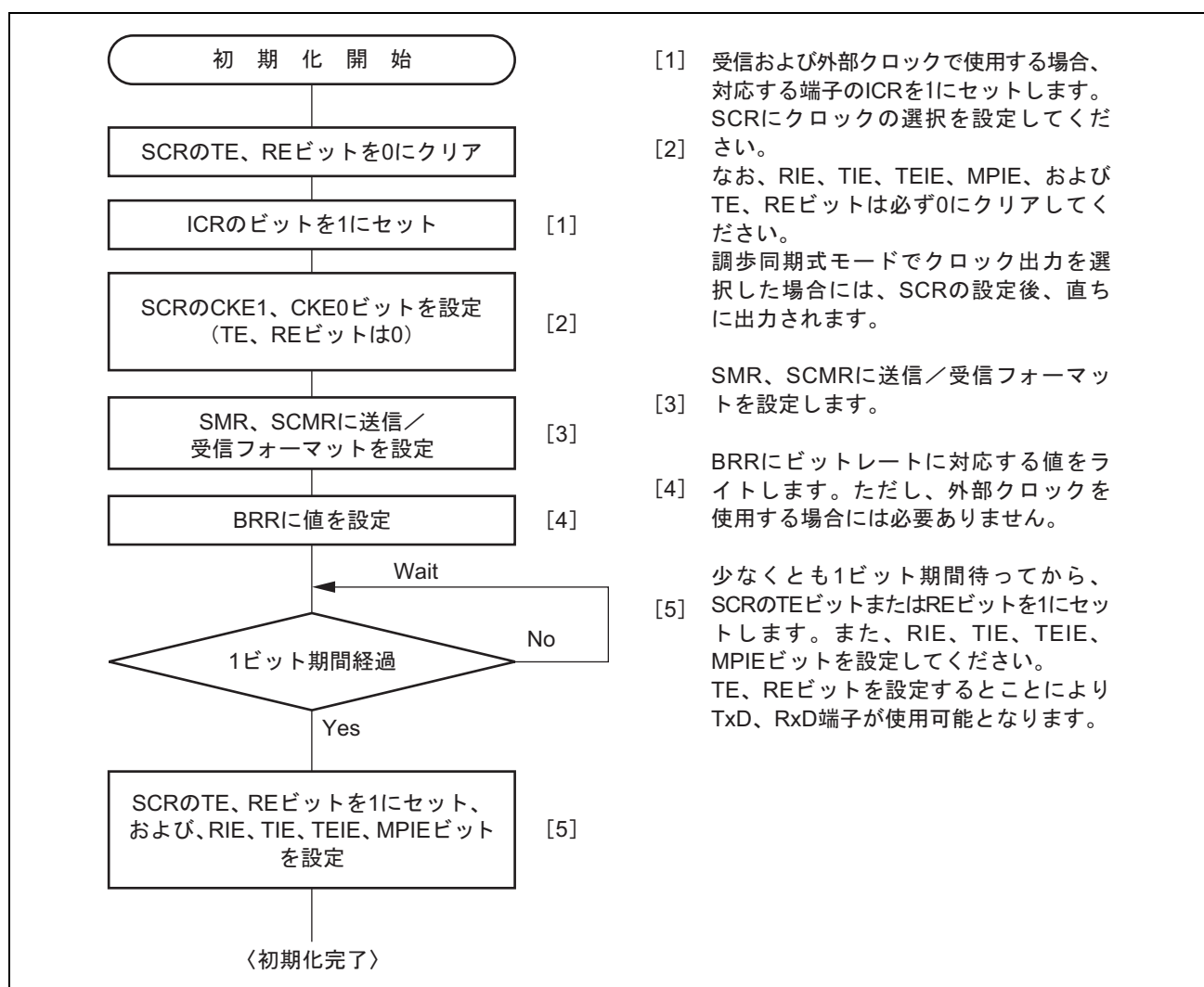
図 17.8 SCI の初期化フローチャートの例
