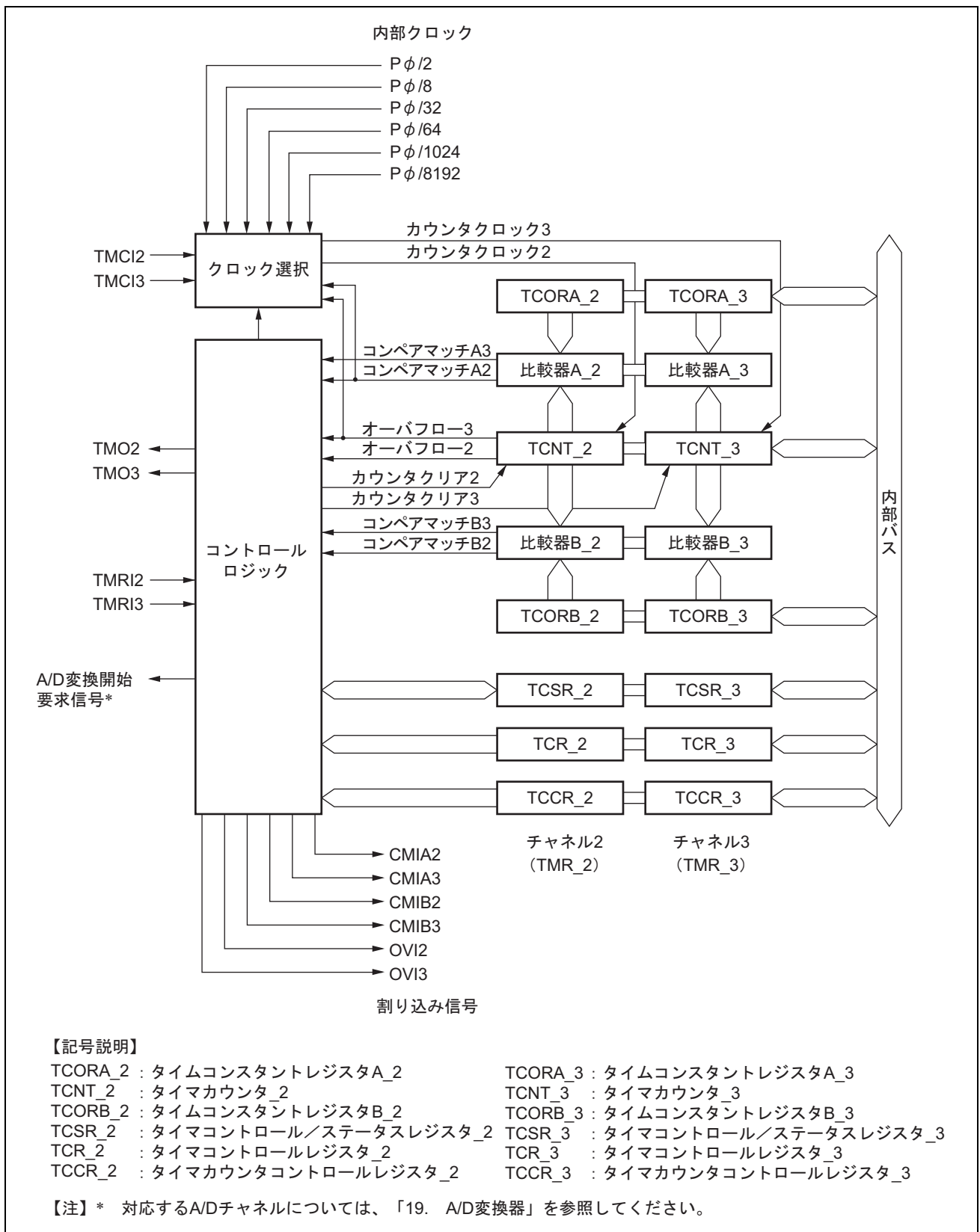
図 15.2 8ビットタイマ (ユニット1) のブロック図
