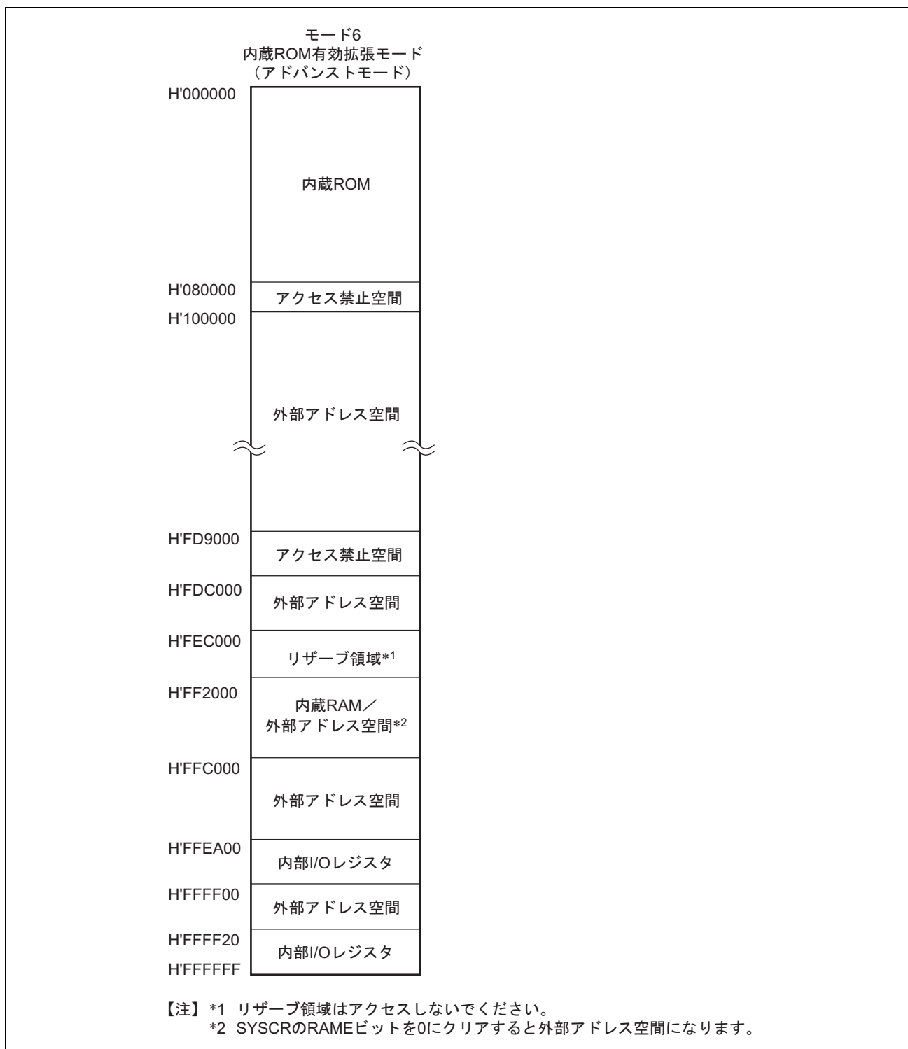
図 3.2 H8SX/1634、1634L の各動作モードのアドレスマップ (2)
