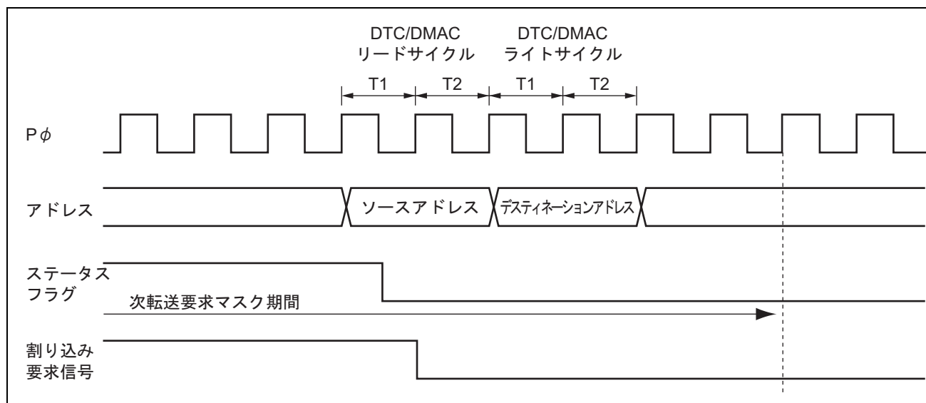
図 13.44 DTC/DMAC の起動によるステータスフラグのクリアタイミング例 (1)
