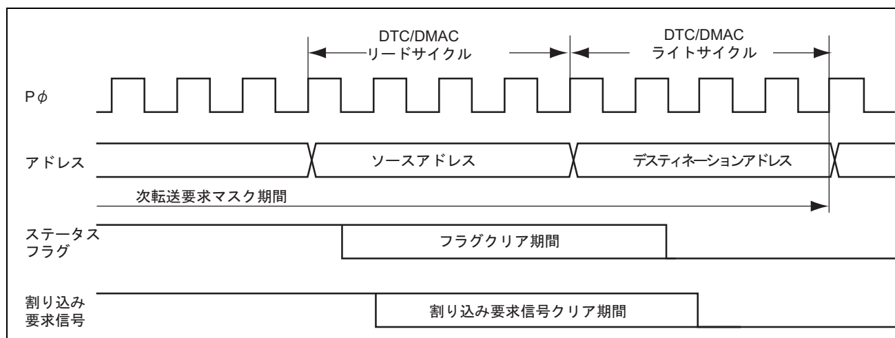
図 13.45 DTC/DMAC の起動によるステータスフラグのクリアタイミング例 (2)
