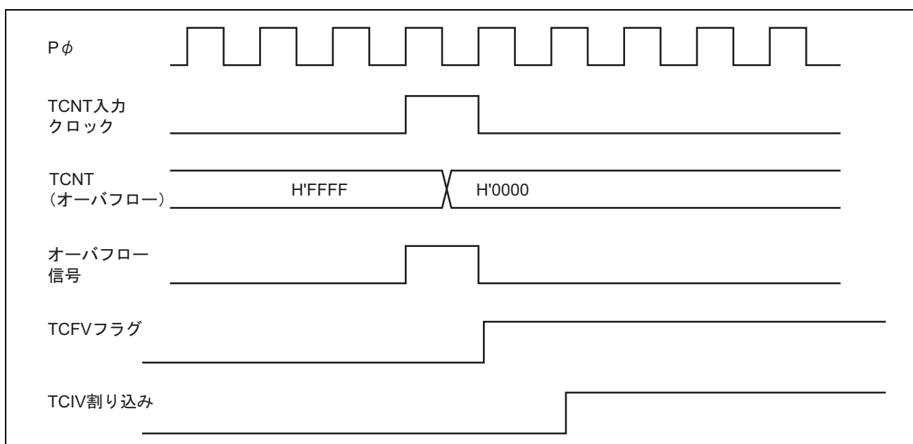
図 13.41 TCIV 割り込みのセットタイミング
