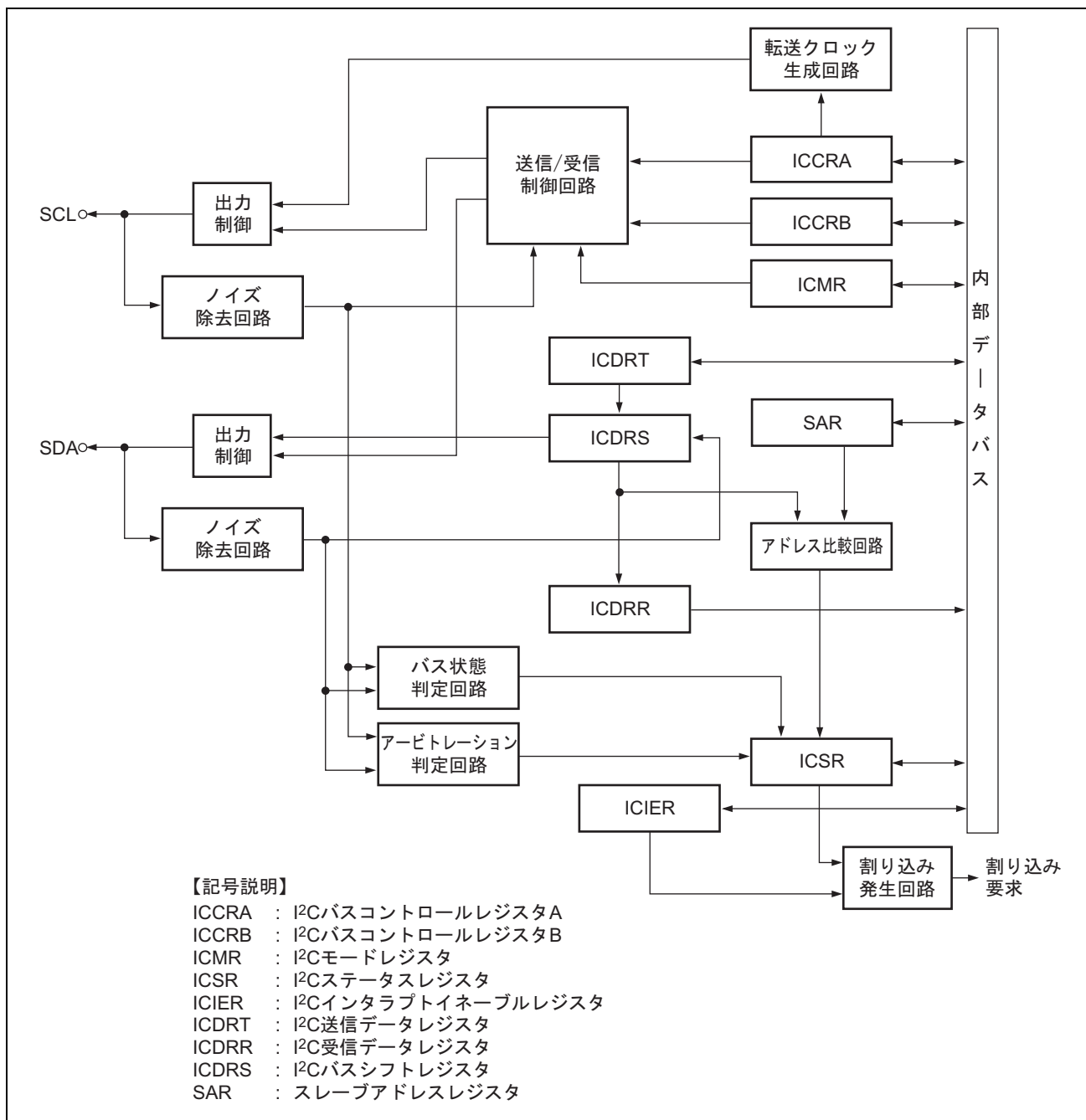
図 18.1 I 2 C バスインタフェース 2 のブロック図
