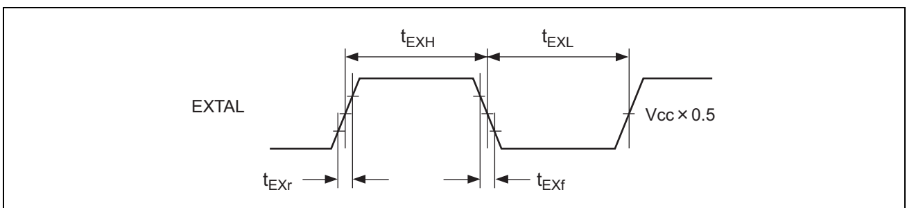
図 27.5 外部入力クロックタイミング
