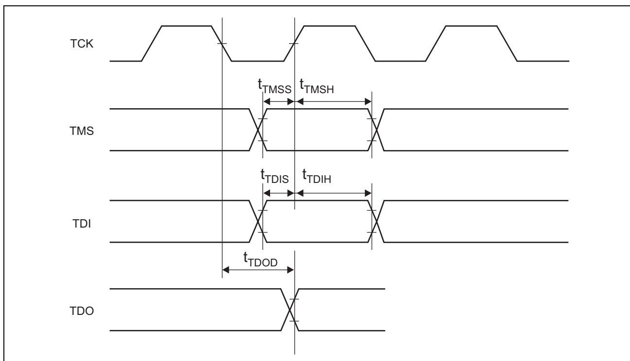
図 27.39 バウンダリスキャン入出力タイミング
