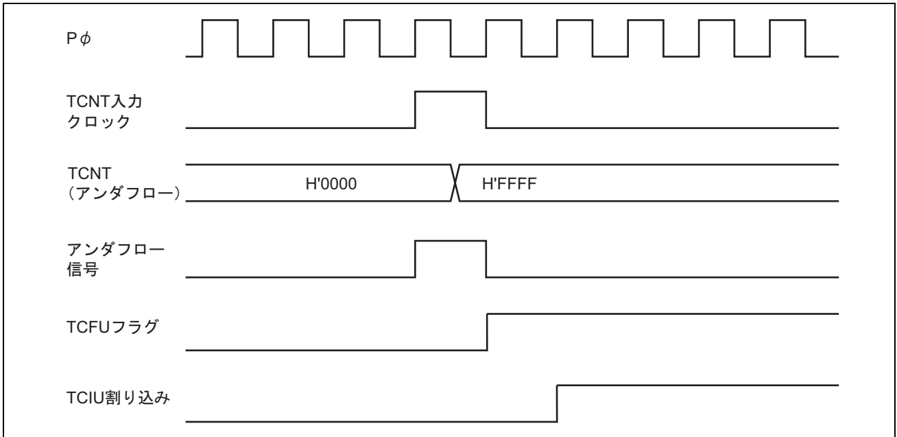
図 13.42 TCIU 割り込みのセットタイミング
