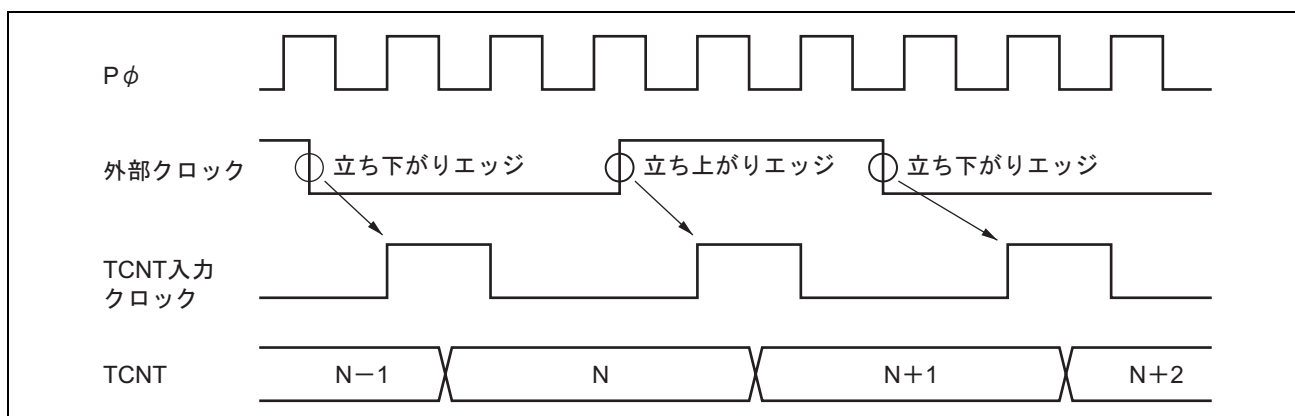
図 13.32 外部クロック動作時のカウントタイミング
