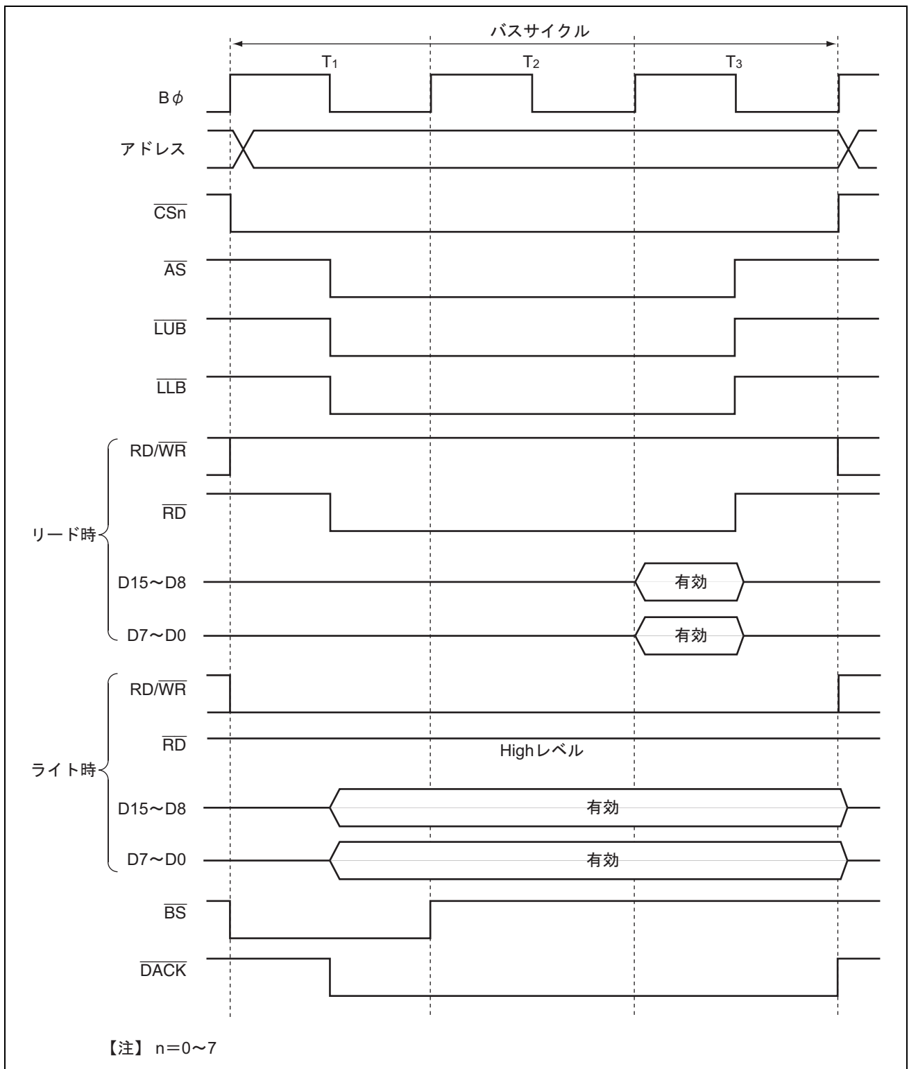
図 9.25 16 ビット 3 ステートアクセス空間のバスタイミング
