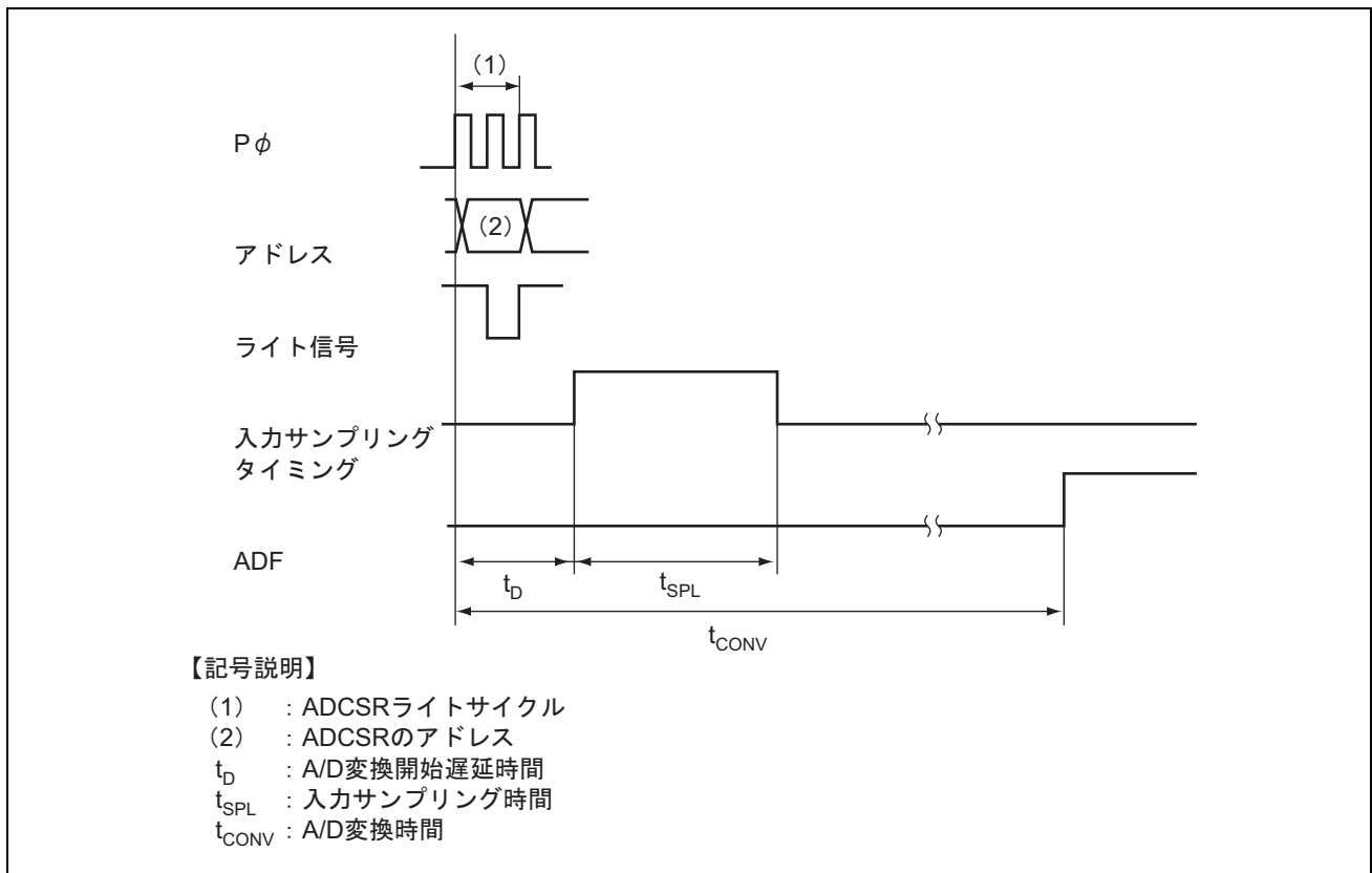
図 19.6 A/D 変換タイミング
