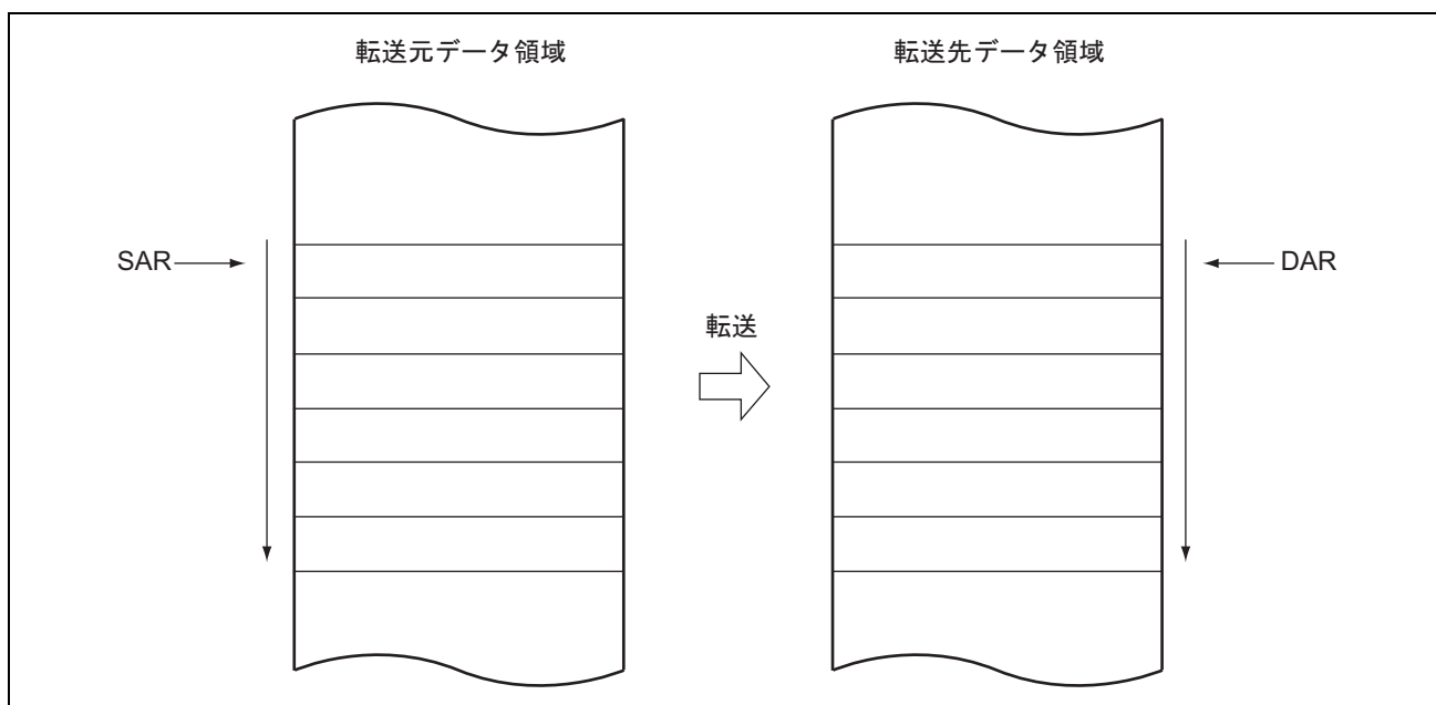
図 11.7 ノーマル転送モードのメモリマップ
