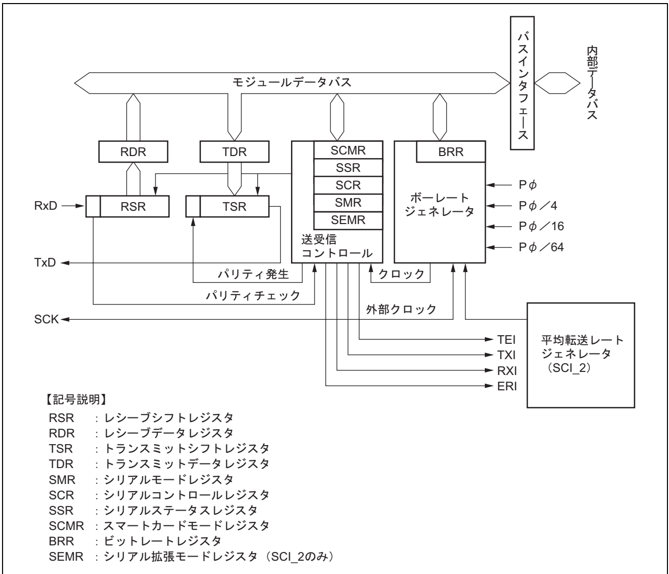
図 17.1 SCI_0、1、2、3、4 のブロック図
