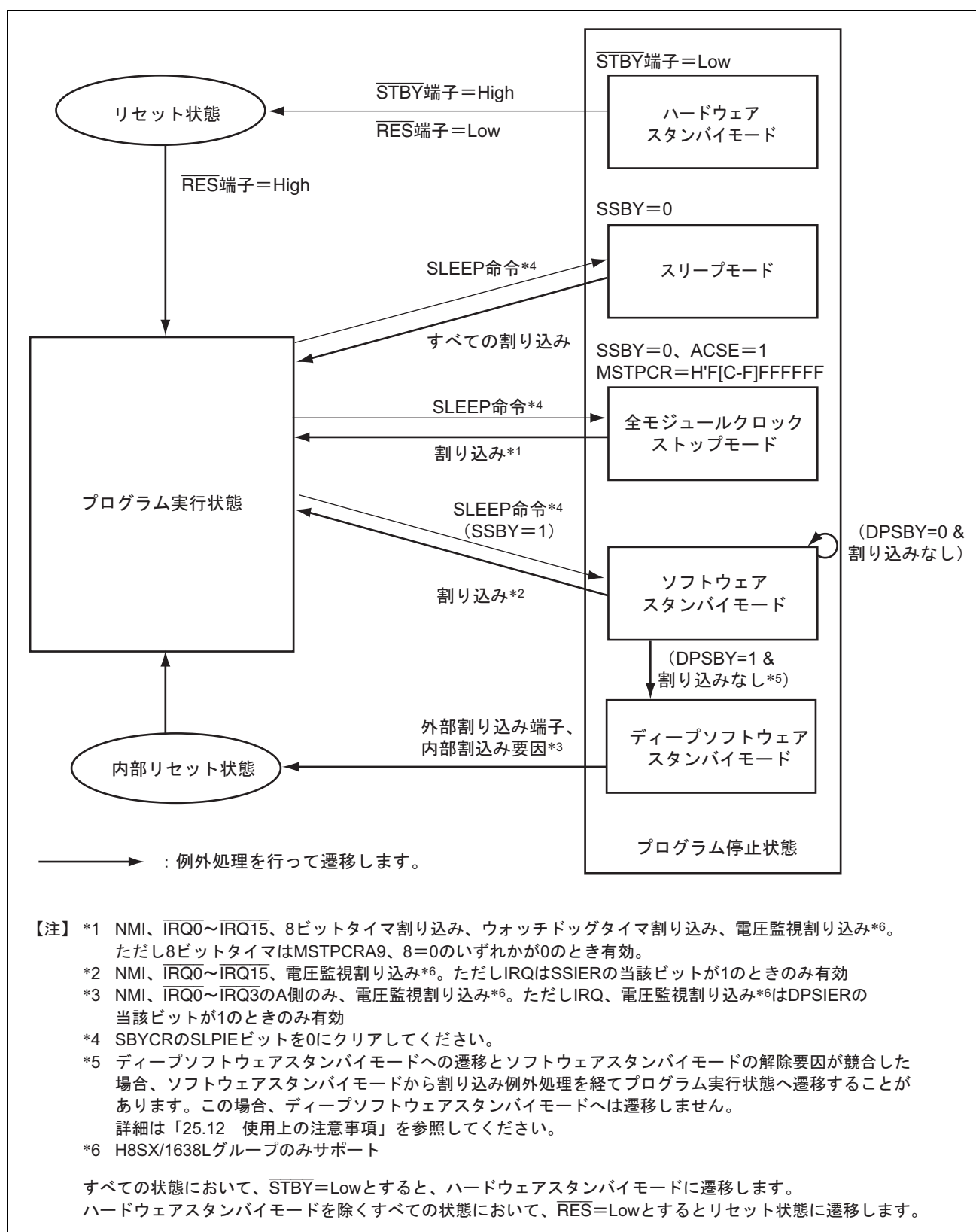
図 25.1 モード遷移
