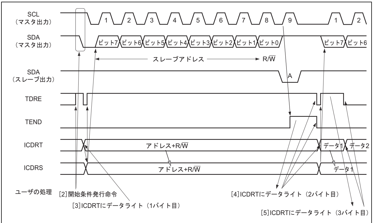
図 18.5 マスタ送信モード動作タイミング 1
