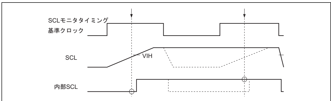
図 18.18 ビット同期回路のタイミング
