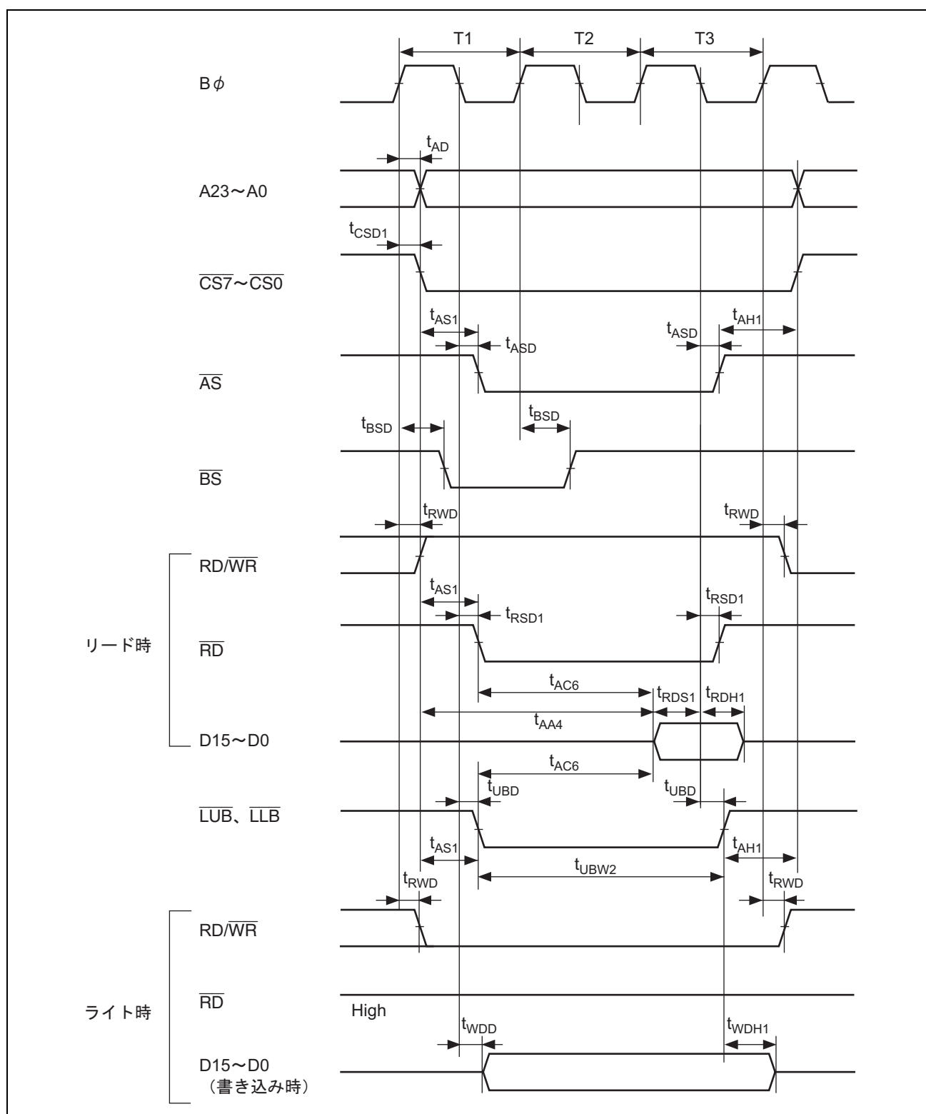
図 27.14 バイト制御 SRAM 3 ステートリード/ライトアクセス
