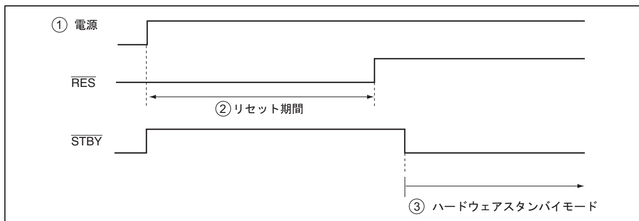
図 25.9 電源投入時のタイミング
