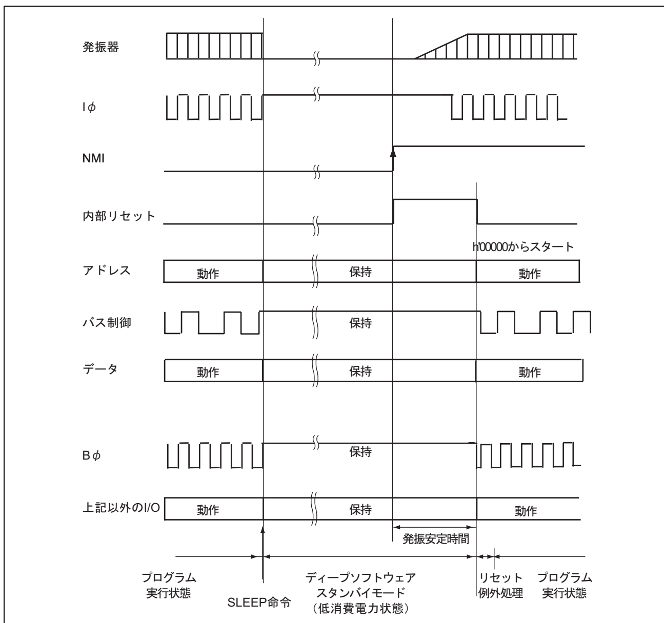
図 25.6 外部拡張モード時のディープソフトウェアスタンバイモードの動作例 (IOKEEP=0、OPE=1 のとき)
