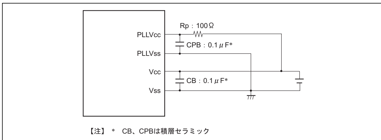
図 24.8 PLL 回路の外付け推奨回路
