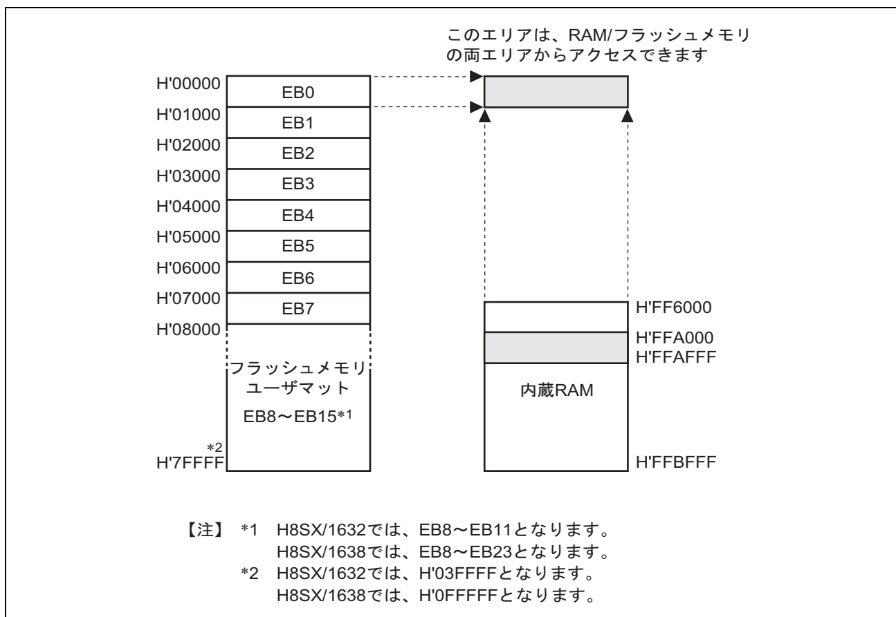
図 22.18 RAM のオーバーラップ動作例 (H8SX/1634)
