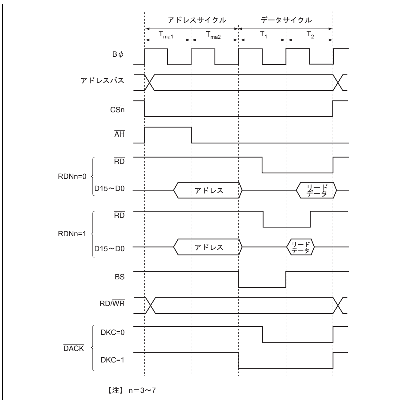
図 9.36 \overline{\text{DACK}} 信号の出力タイミング
