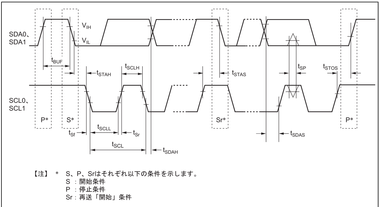
図 27.36 I 2 C バスインタフェース 2 入出力タイミング【オプション】
