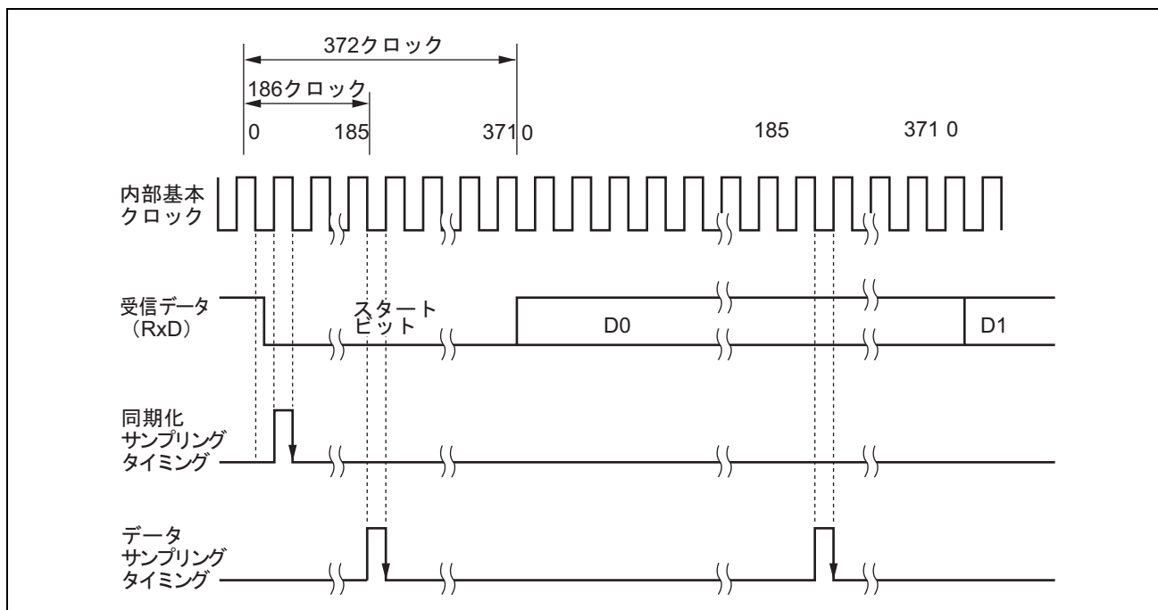
図 17.28 スマートカードインタフェースモード時の受信データサンプリングタイミング (372 倍のクロック使用時)
