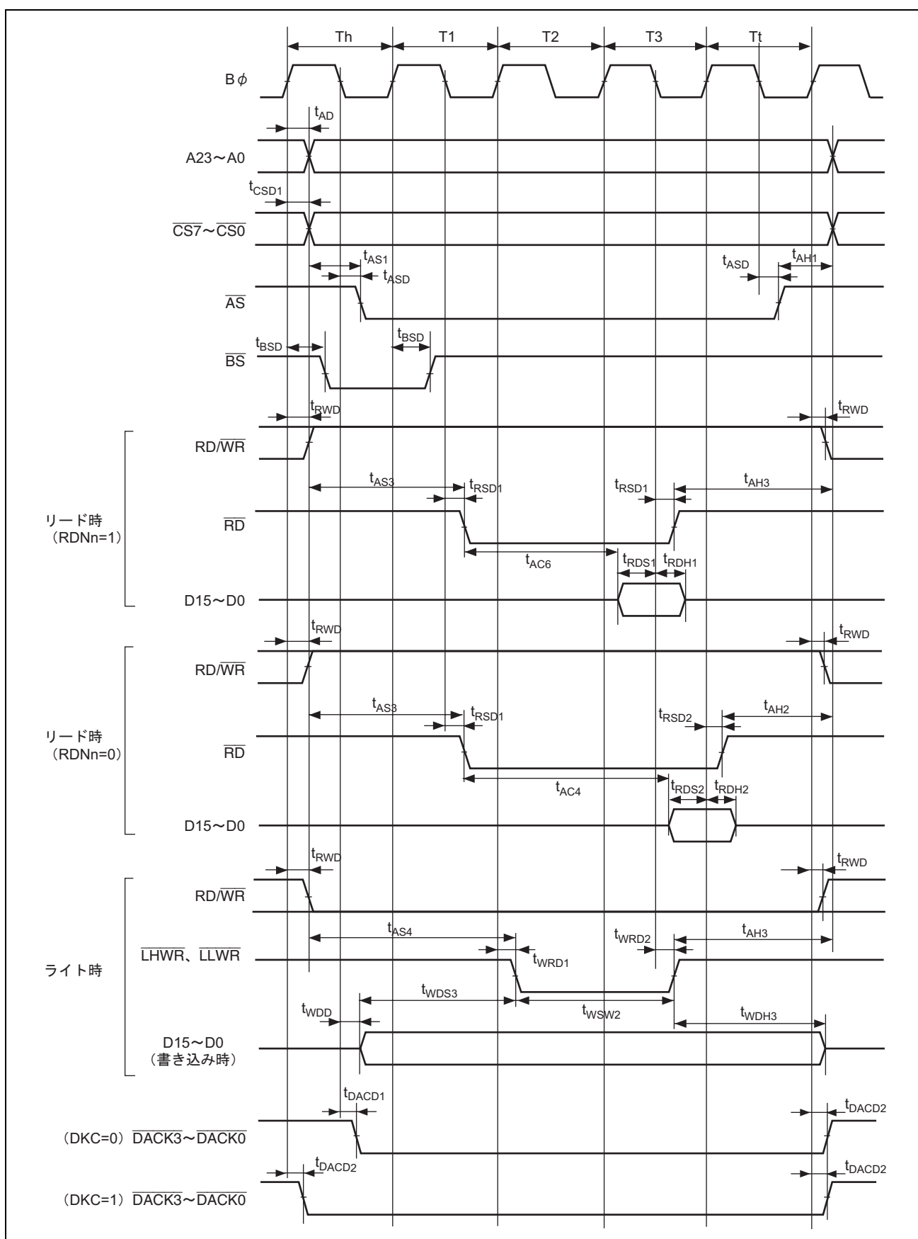
図 27.12 基本バスタイミング/3 ステートアクセス (CS アサート期間延長)
