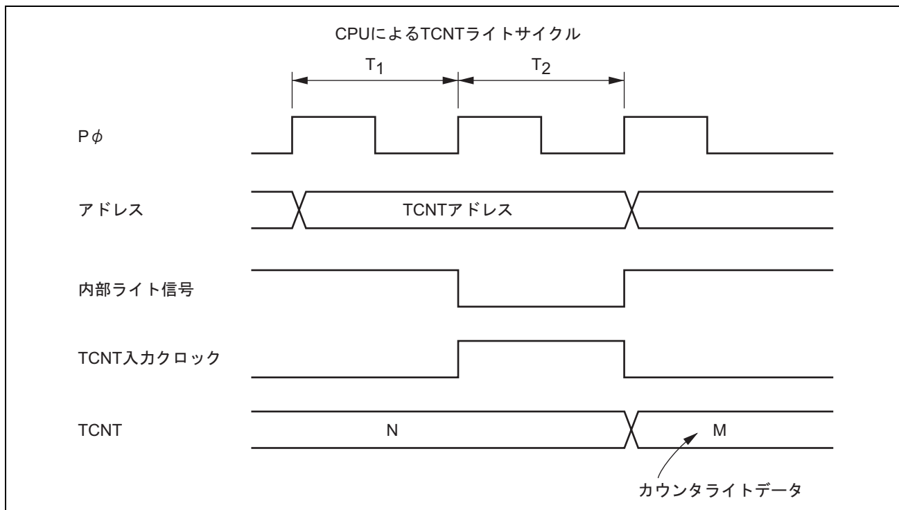
図 15.16 TCNT のライトとカウントアップの競合
