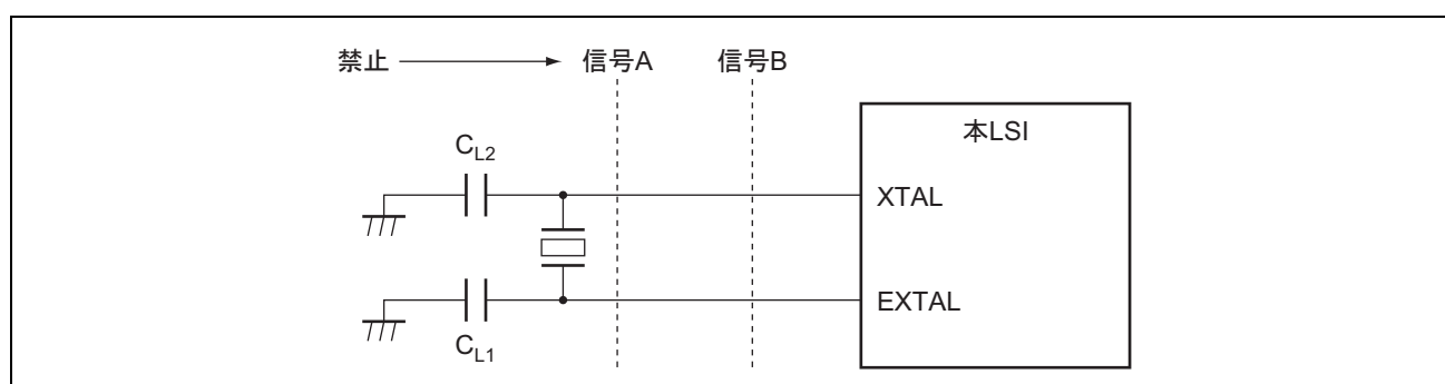
図 24.7 発振回路部のボード設計に関する注意事項
