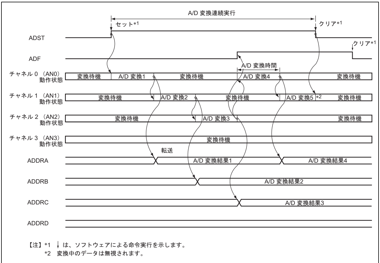
図 19.4 A/D 変換器の動作例 (連続スキャンモード、AN0~AN2 の 3 チャンネル選択時)
