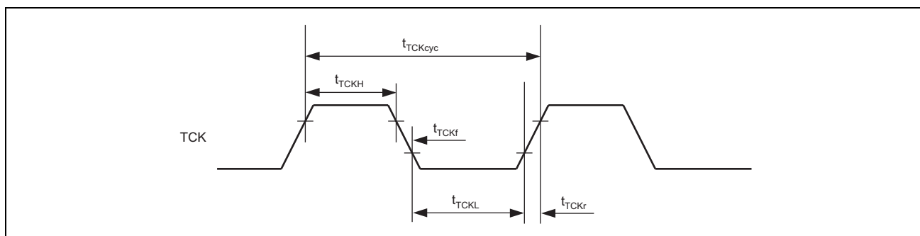
図 27.37 バウンダリスキャン TCK タイミング
