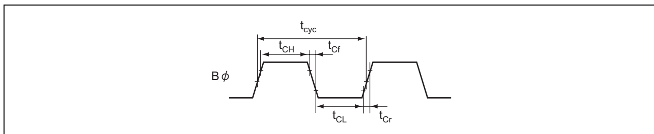
図 27.2 外部バスクロックタイミング
