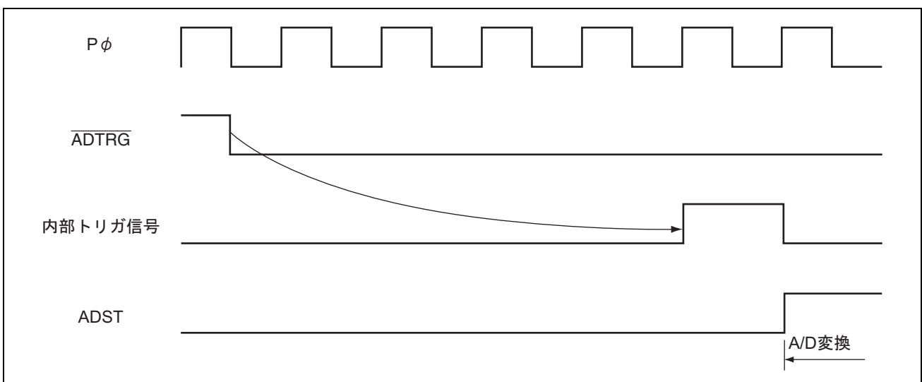
図 19.8 外部トリガ入力タイミング (ユニット同時起動時 : TRGS1、TRGS0、EXTRGS=B'111)
