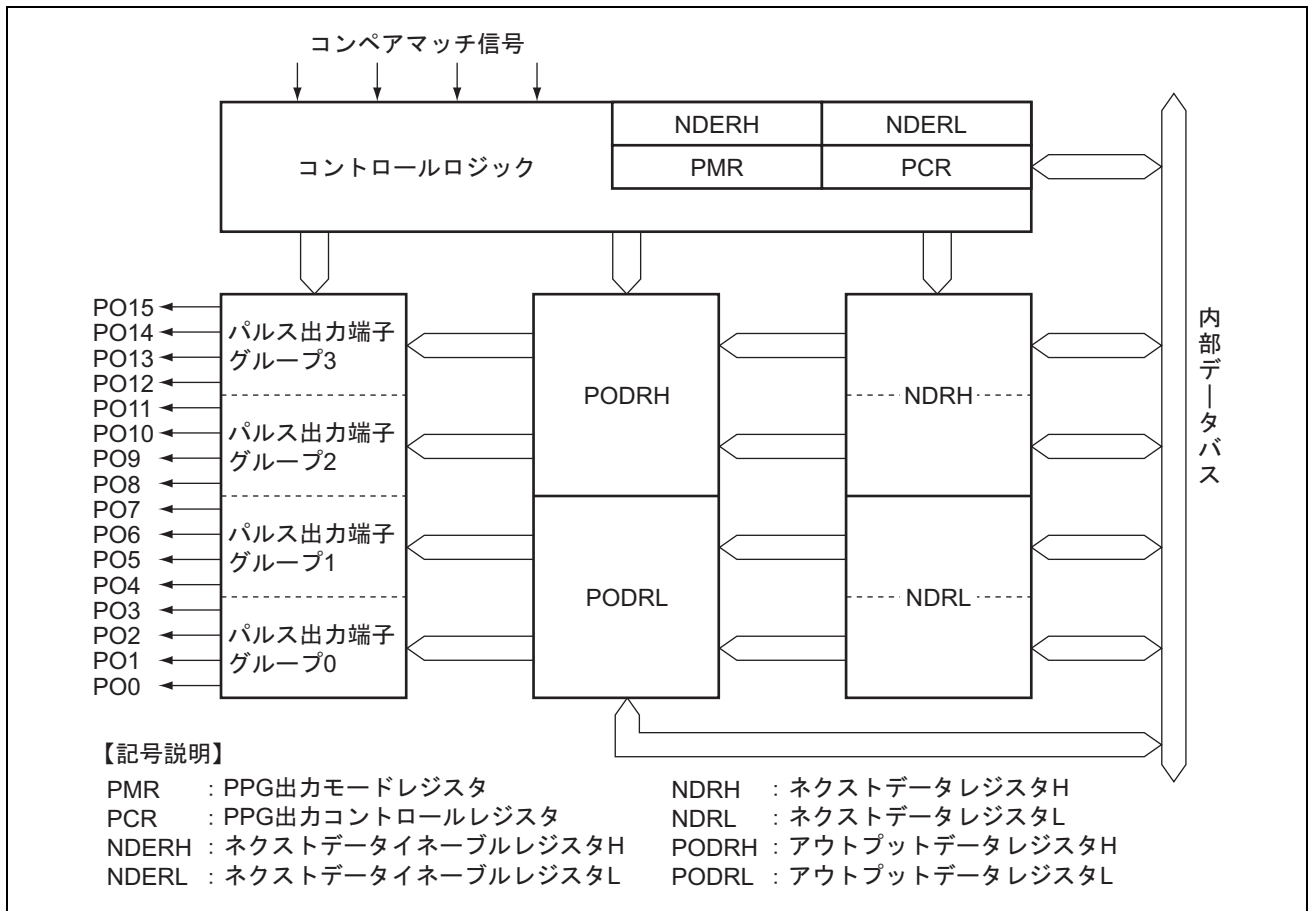
図 14.1 PPG (ユニット0) のブロック図
