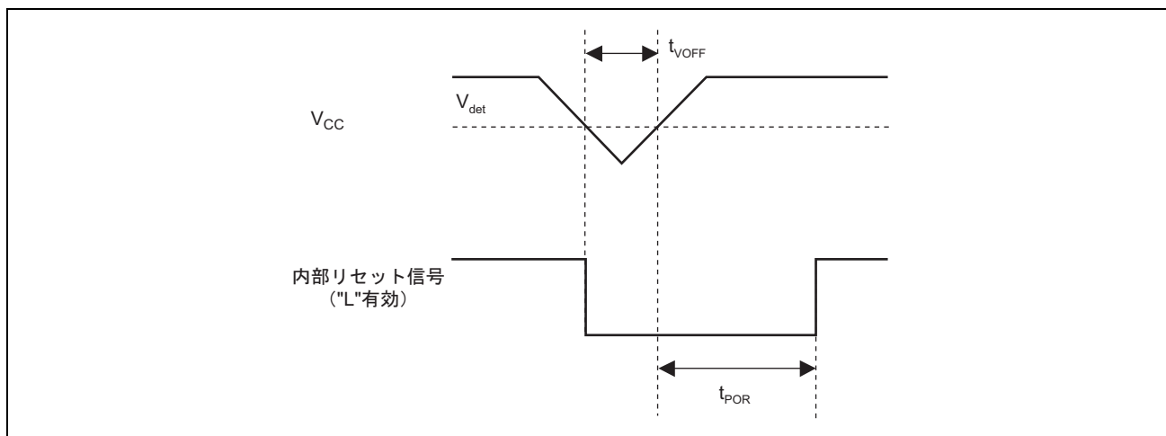
図 27.41 電圧検出回路タイミング
