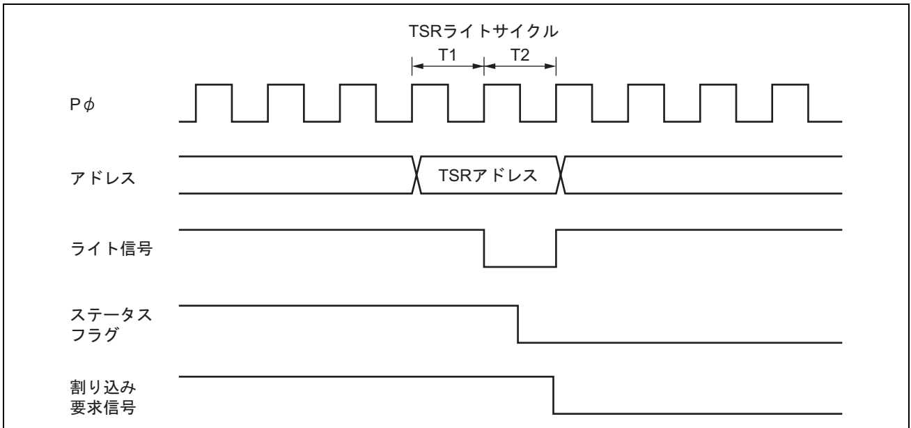
図 13.43 CPUによるステータスフラグのクリアタイミング
