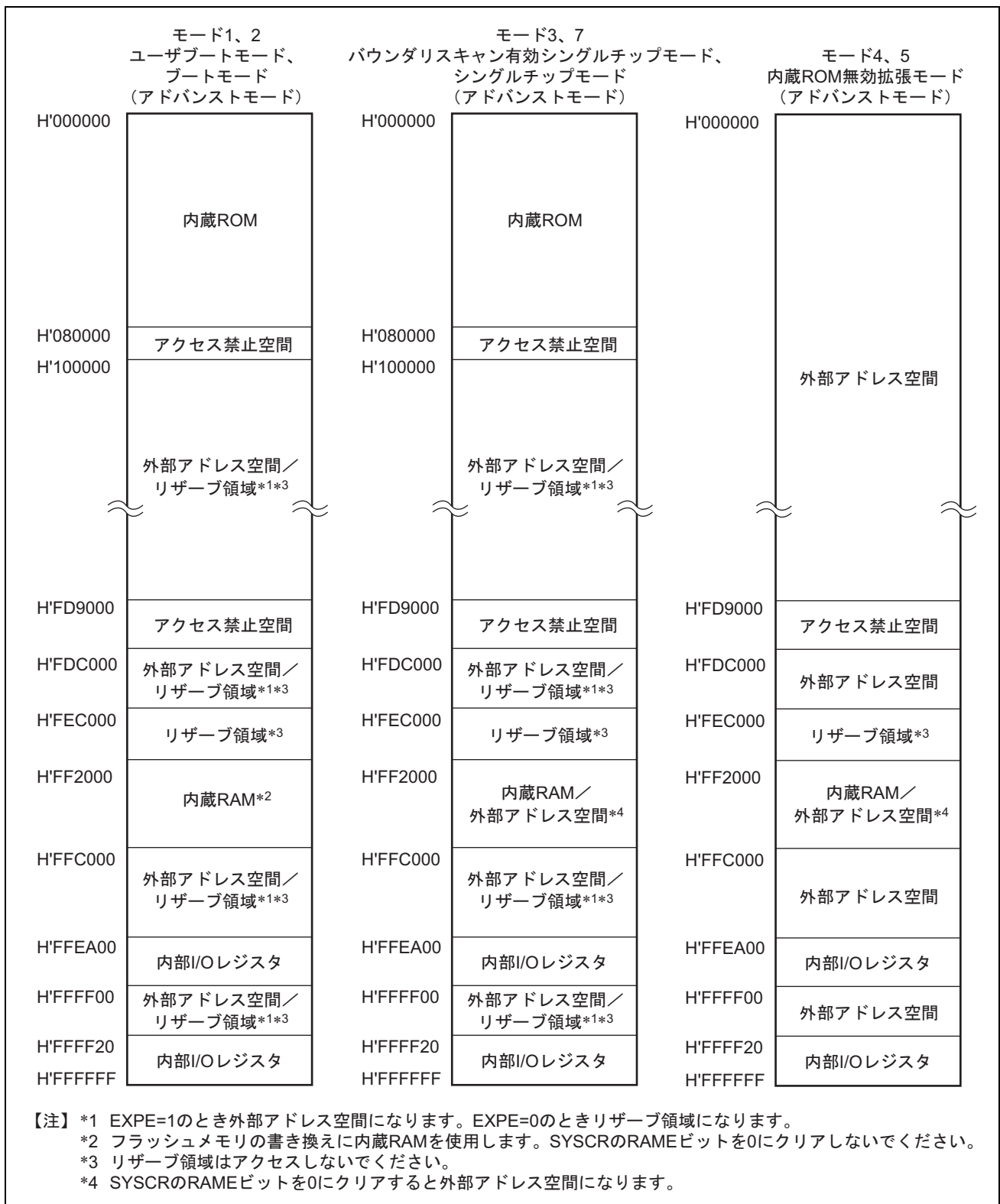
図 3.2 H8SX/1634、1634L の各動作モードのアドレスマップ (1)
