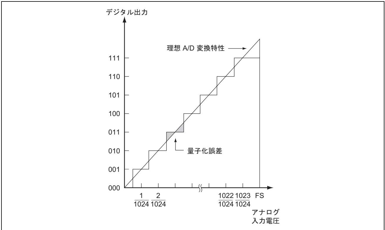
図 19.9 A/D 変換精度の定義
