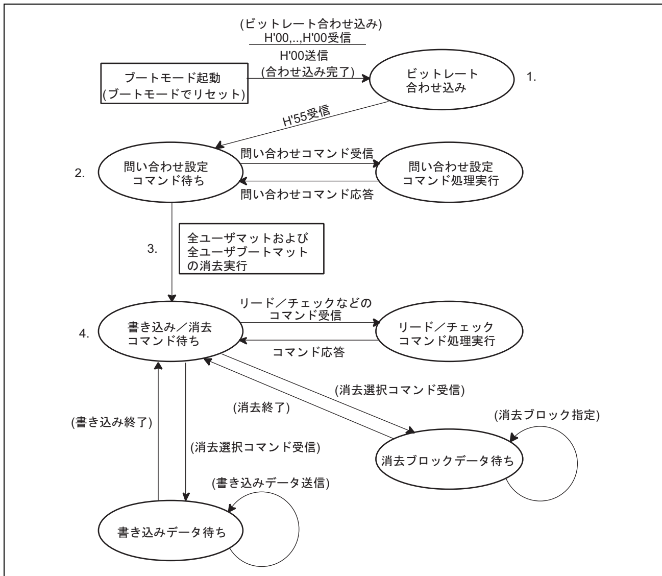
図 22.8 ブートモードの状態遷移図
