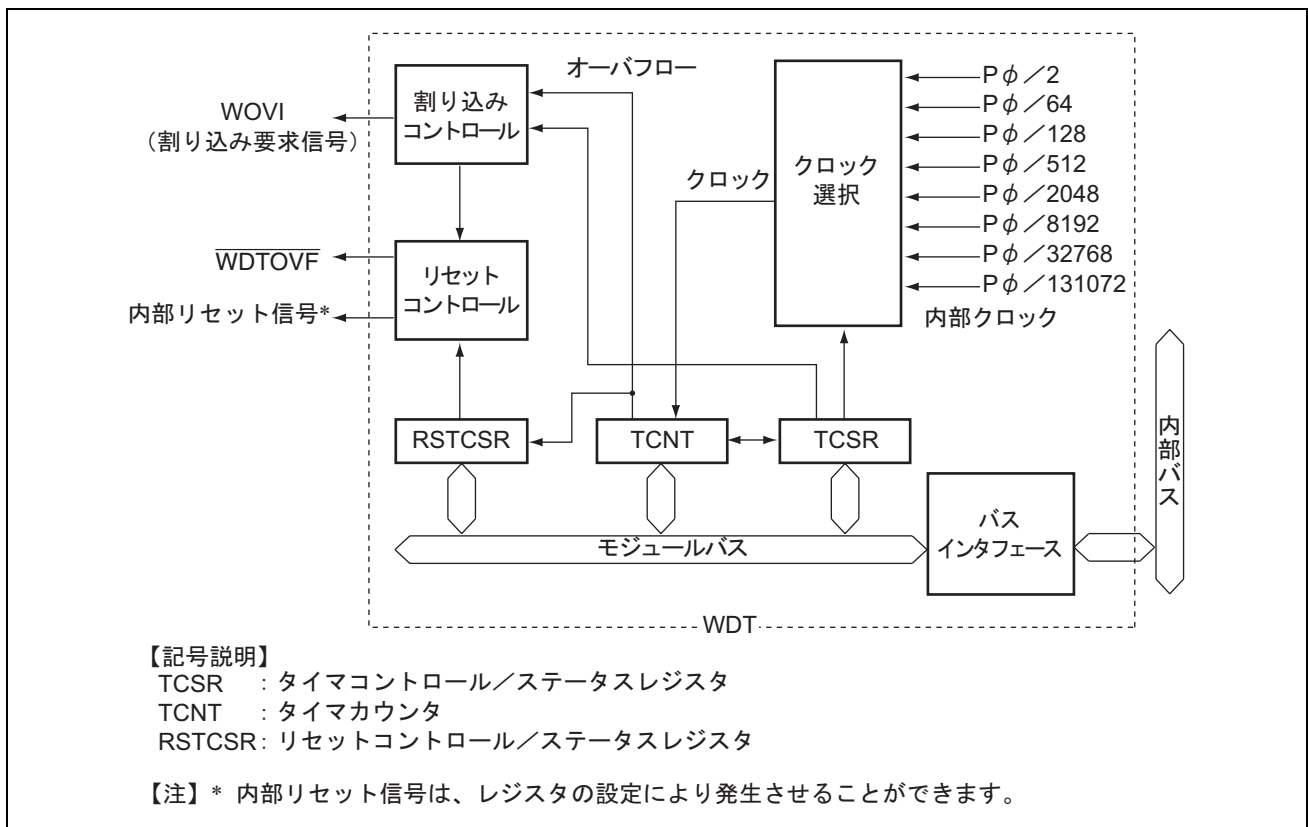
図 16.1 WDT のブロック図
