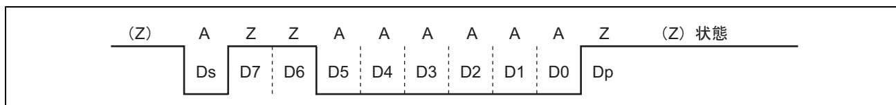
図 17.27 インバースコンベンション (SDIR=SINV=O/E=1)
