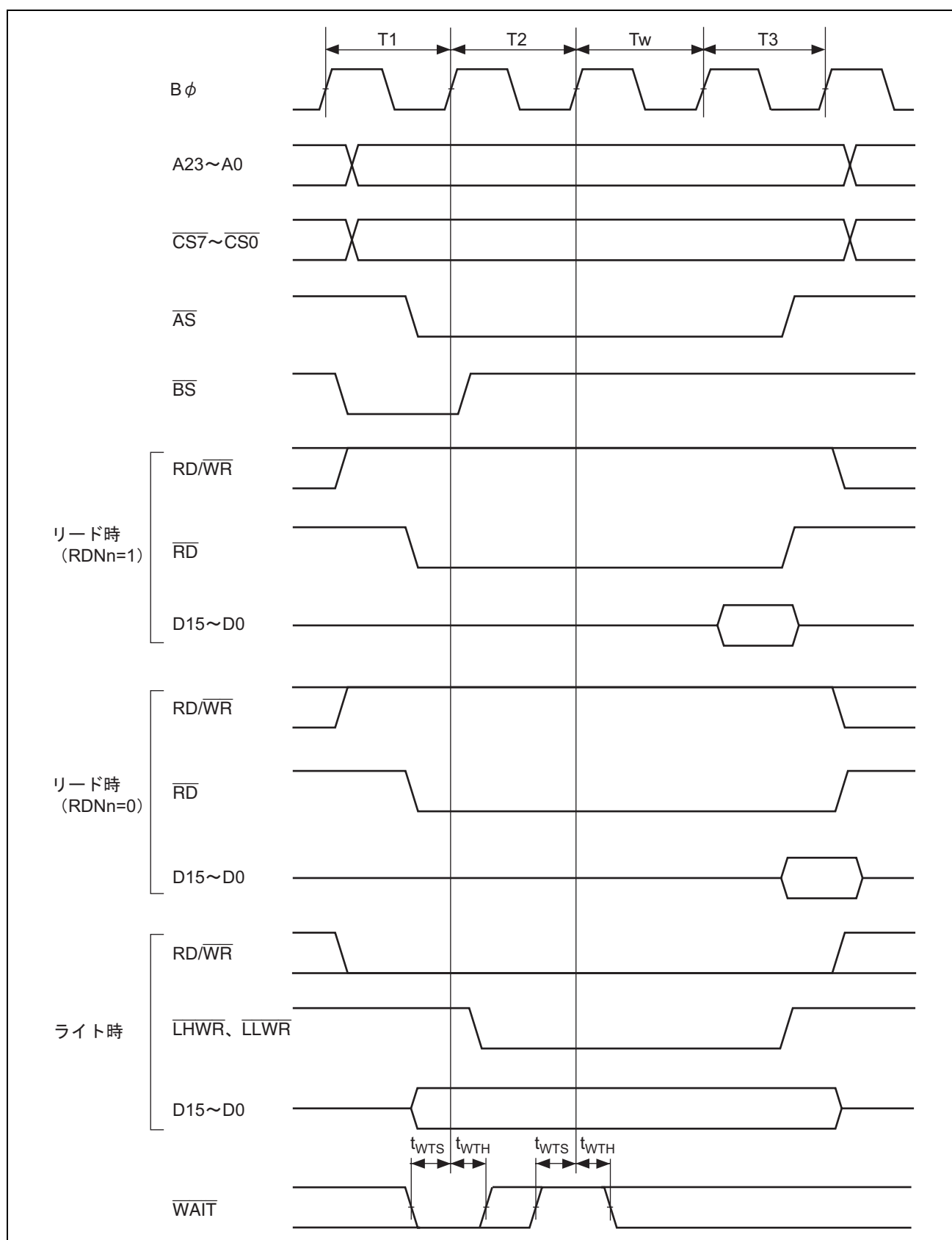
図 27.10 基本バスタイミング/3 ステートアクセス 1 ウェイト
