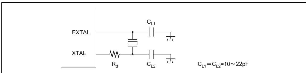
図 24.2 水晶発振子の接続例
