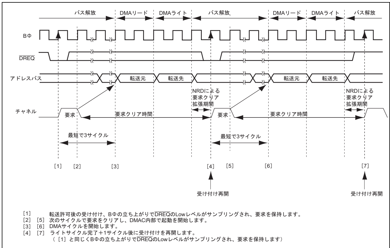
図 10.33 NRD=1 のときの \overline{\text{DREQ}} Low レベル起動時のノーマル転送モードの転送例
