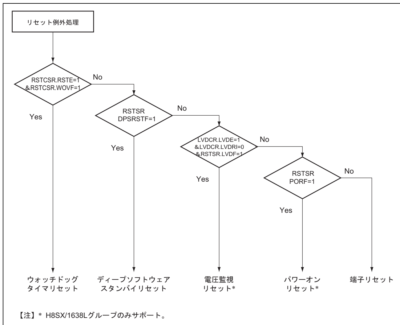
図 4.3 リセット発生要因判定フロー例
