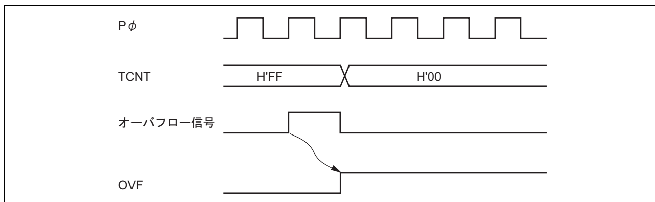
図 15.14 OVF フラグのセットタイミング
