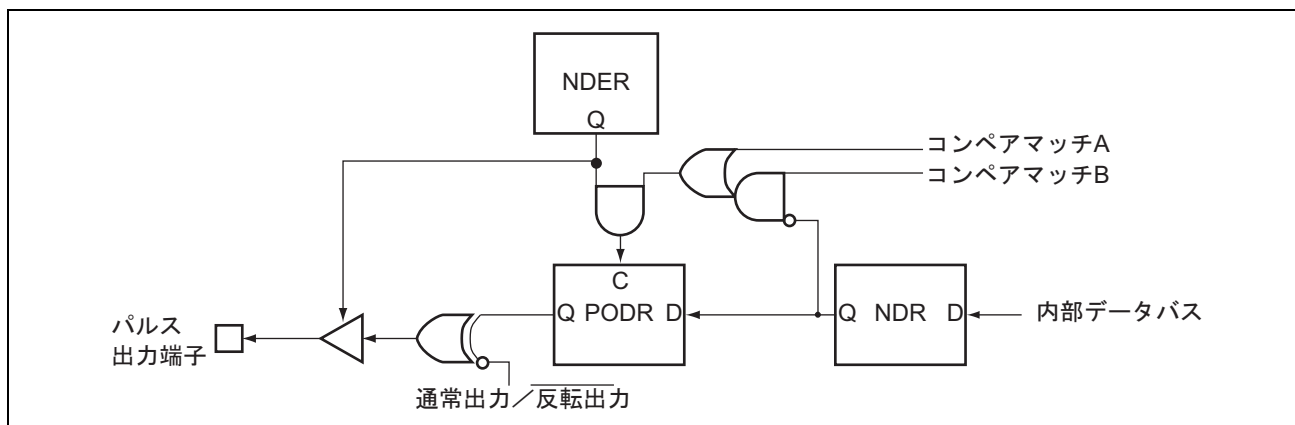
図 14.8 パルス出力ノンオーバーラップ動作
