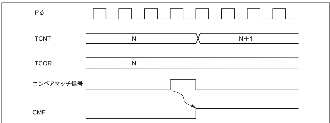
図 15.9 コンペアマッチ時の CMF フラグのセットタイミング
