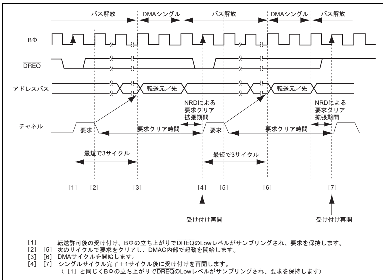
図 10.38 \overline{\text{NRD}}=1 のときの \overline{\text{DREQ}} Low レベル起動時のシングルアドレスモードの転送例
