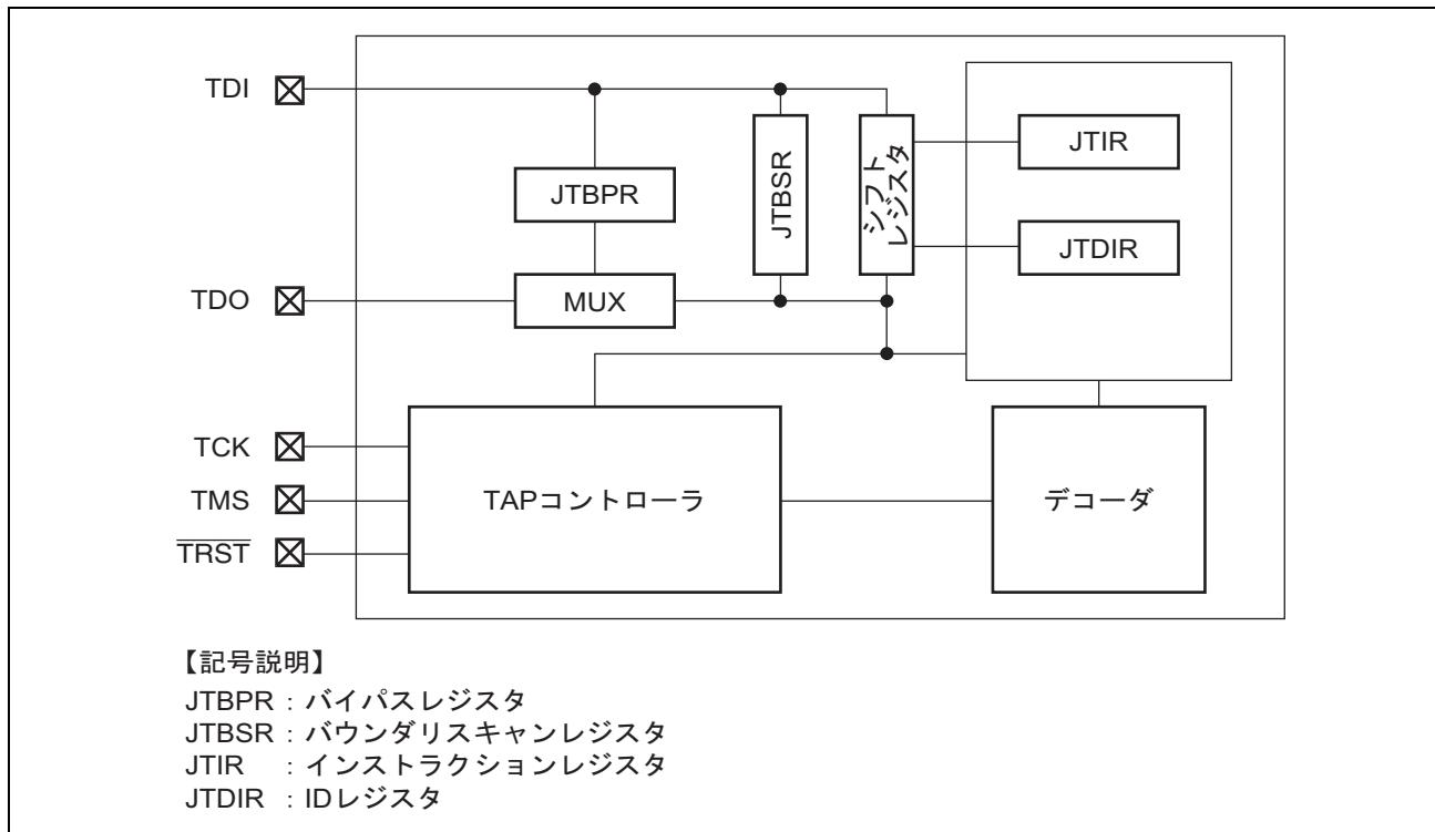
図 23.1 JTAG ブロック図
