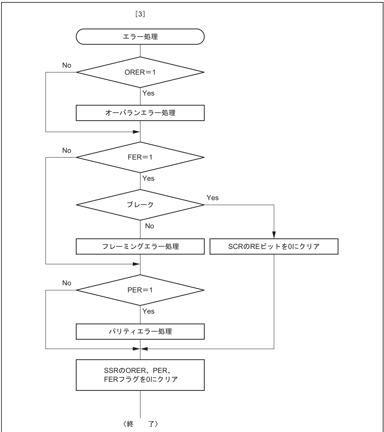
図 17.12 シリアル受信のフローチャートの例 (2)
