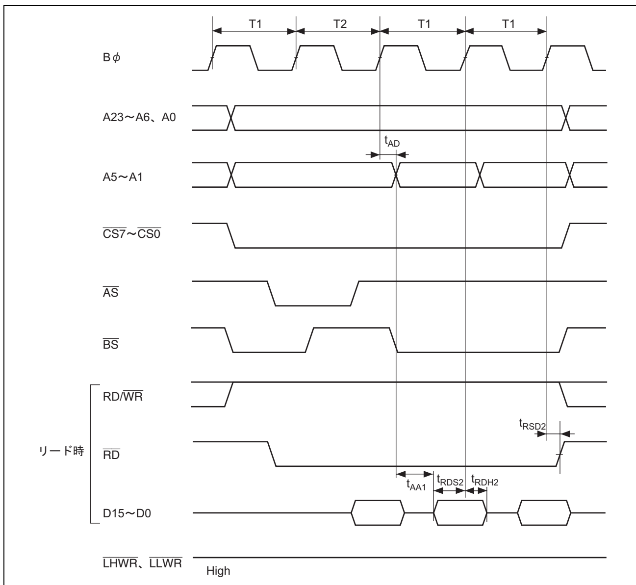
図 27.15 バースト ROM アクセスタイミング/1 ステートバーストアクセス
