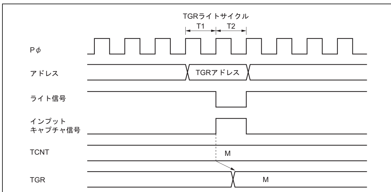
図 13.52 TGRのライトと入力キャプチャの競合
