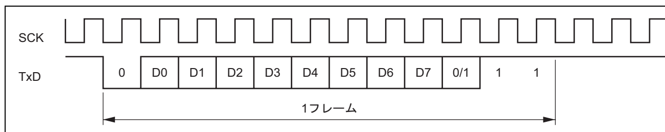
図 17.7 出力クロックと送信データの位相関係（調歩同期式モード）
