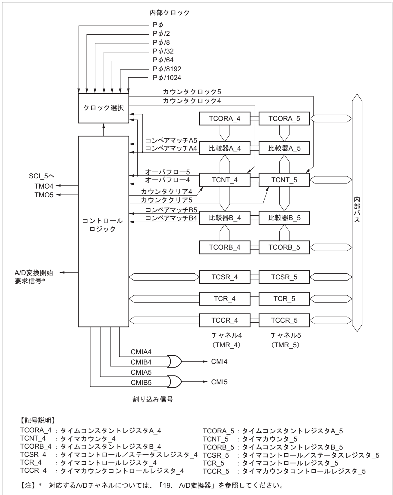
図 15.3 8ビットタイマ (ユニット2) のブロック図
