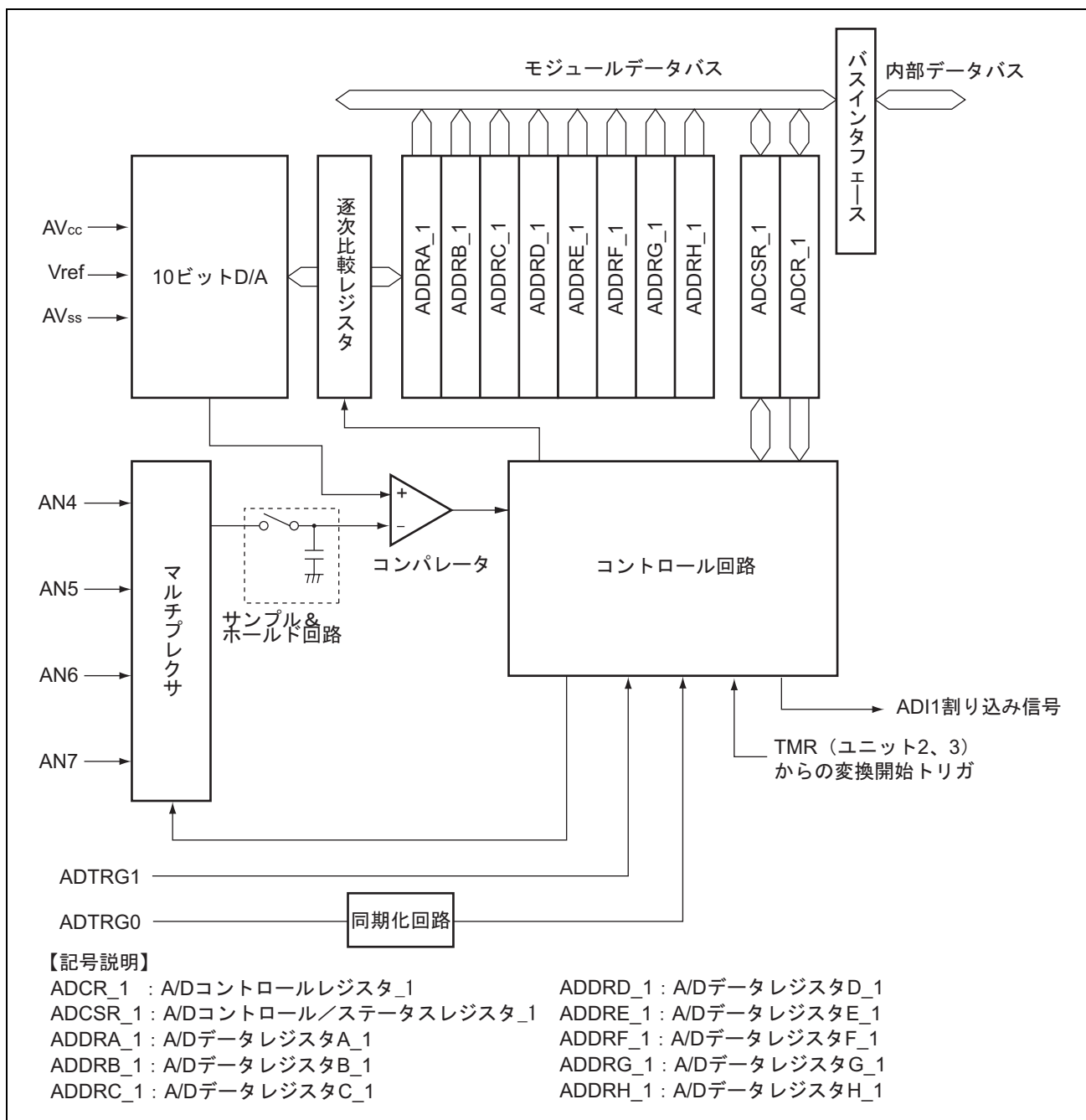
図 19.2 A/D 変換器 (ユニット 1/AD_1) のブロック図
