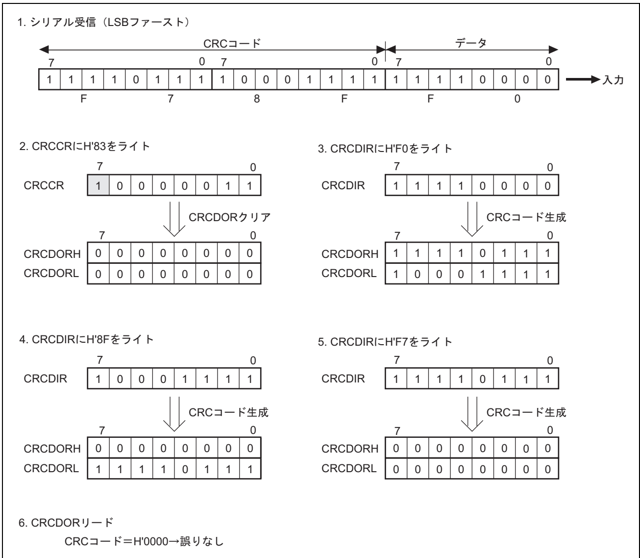
図 17.46 LSB ファーストでのデータ受信
