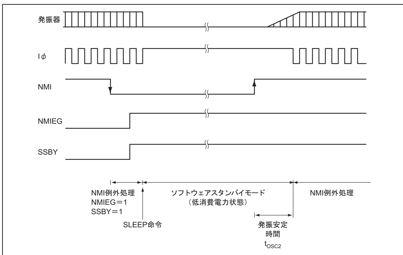
図 25.2 ソフトウェアスタンバイモードの応用例
