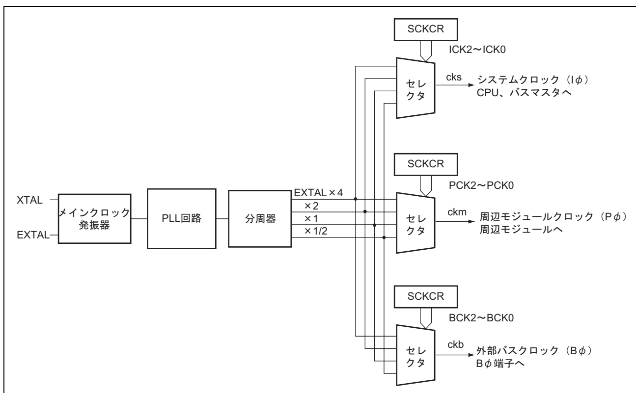
図 24.1 クロック発振器のブロック図
