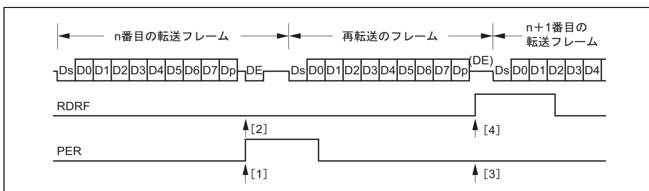
図 17.32 SCI 受信モードの場合の再転送動作
