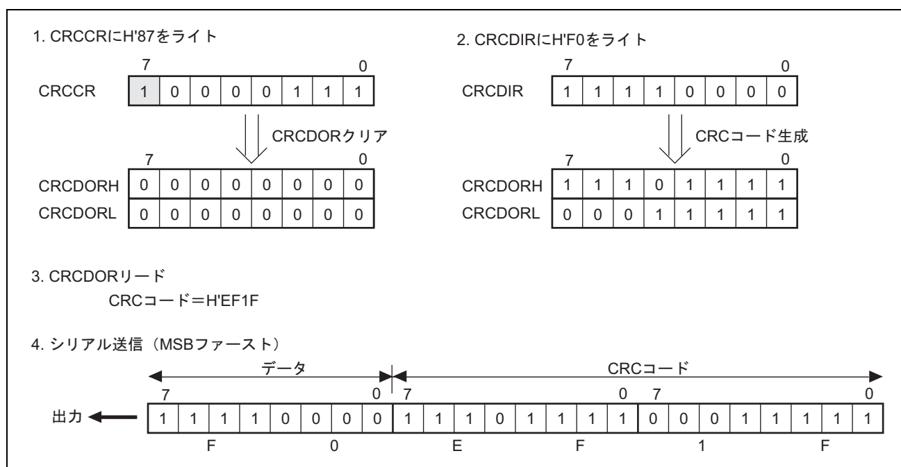
図 17.45 MSB ファーストでのデータ送信
