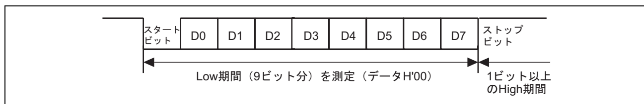
図 22.7 ビットレートの自動合わせ込み
