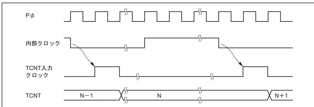
図 15.7 内部クロック動作時のカウントタイミング
