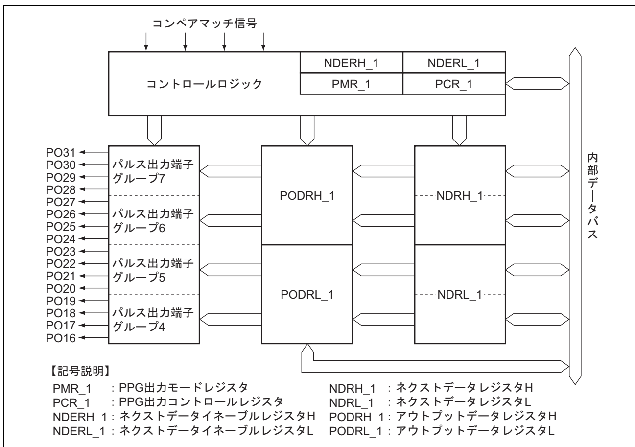
図 14.2 PPG (ユニット1) のブロック図
