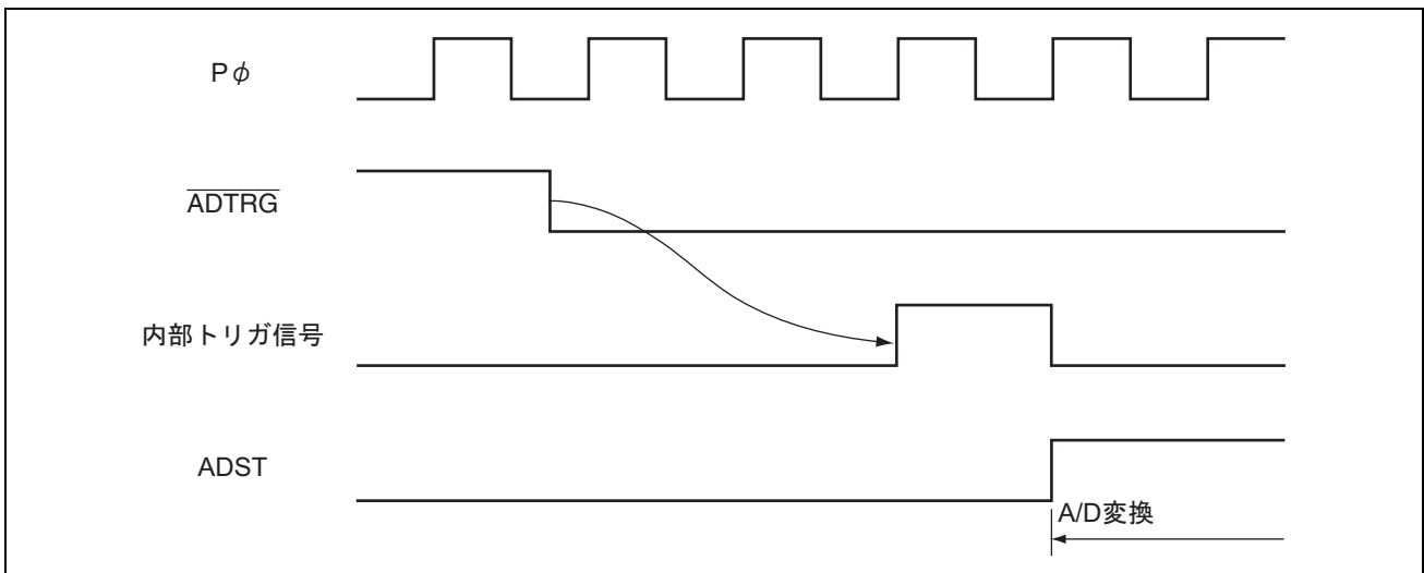
図 19.7 外部トリガ入力タイミング (TRGS1、TRGS0、EXTRGS≠B'111)
