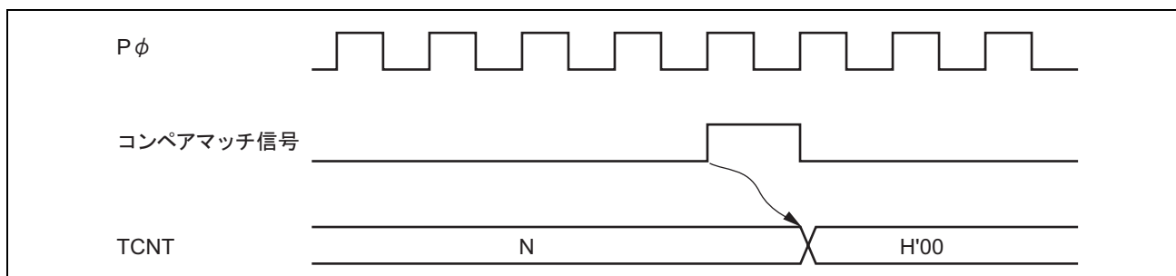
図 15.11 コンペアマッチによるカウンタクリアタイミング
