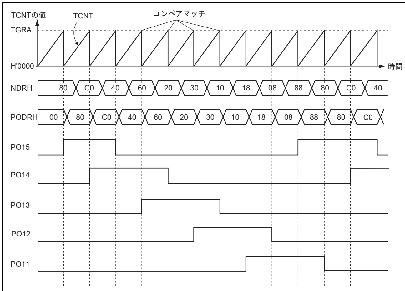
図 14.7 パルス出力通常動作例 (5相パルス出力例)
