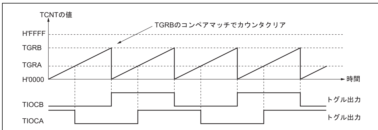
図 13.8 トグル出力の動作例
