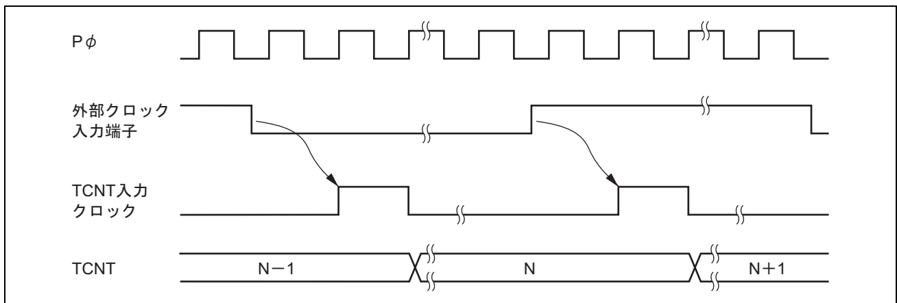
図 15.8 外部クロック動作時のカウントタイミング
