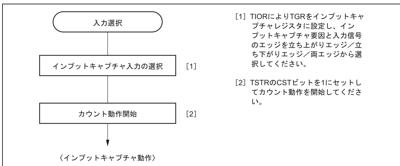
図 13.9 インพุットキャプチャ動作の設定例
