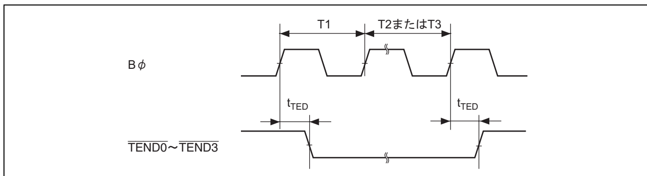
図 27.22 DMAC、 \overline{\text{TEND}} 出力タイミング
