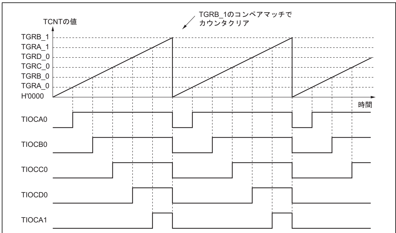
図 13.23 PWM モードの動作例 (2)
