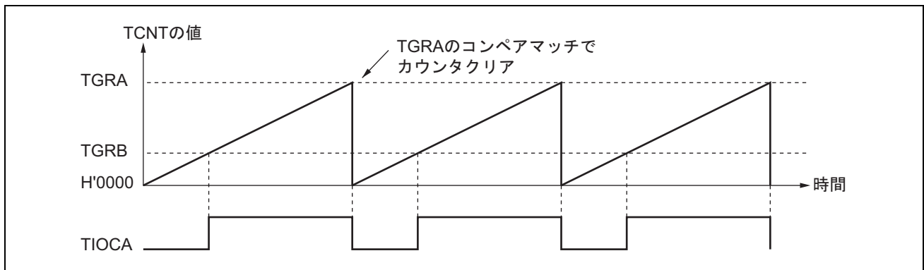
図 13.22 PWM モードの動作例 (1)
