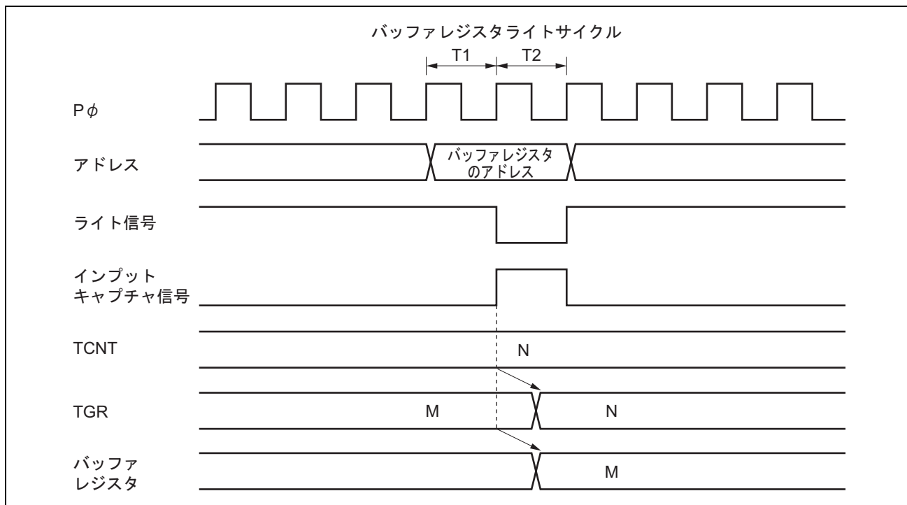
図 13.53 バッファレジスタのライトとインプットキャプチャの競合
