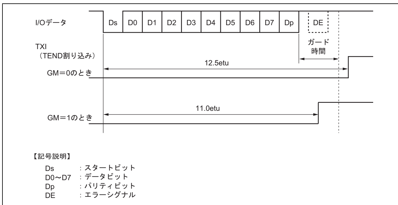
図 17.30 送信動作時の TEND フラグ発生タイミング
