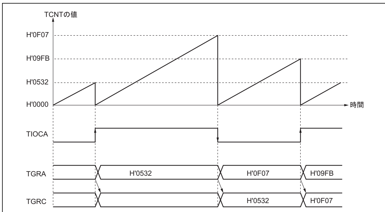
図 13.17 バッファ動作例 (2)
