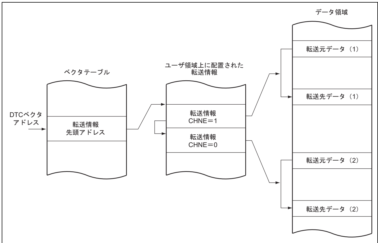
図 11.10 チェイン転送の動作
