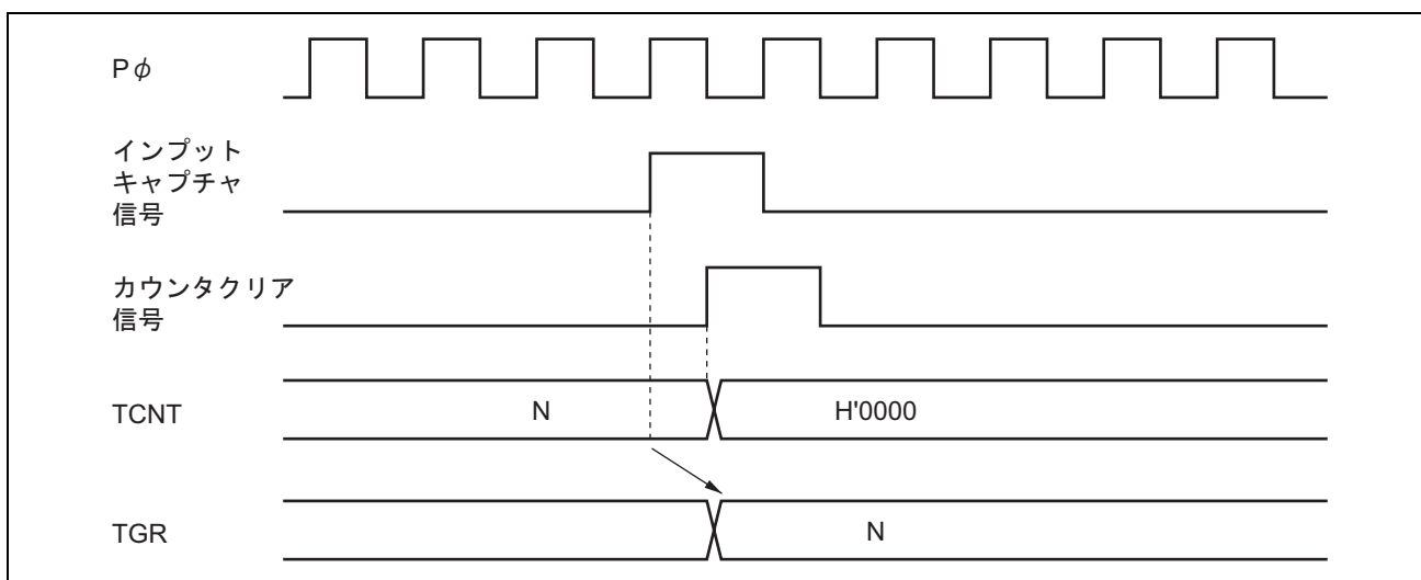
図 13.36 カウンタクリアタイミング (インプットキャプチャ)
