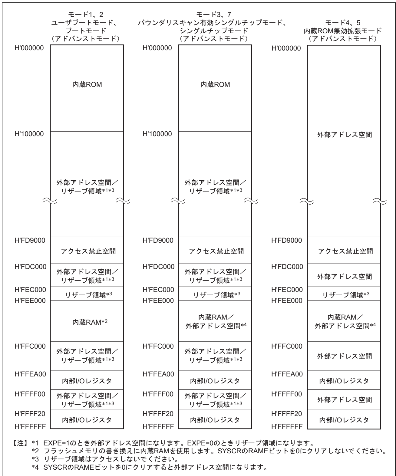
図 3.1 H8SX/1638、1638L の各動作モードのアドレスマップ (1)
