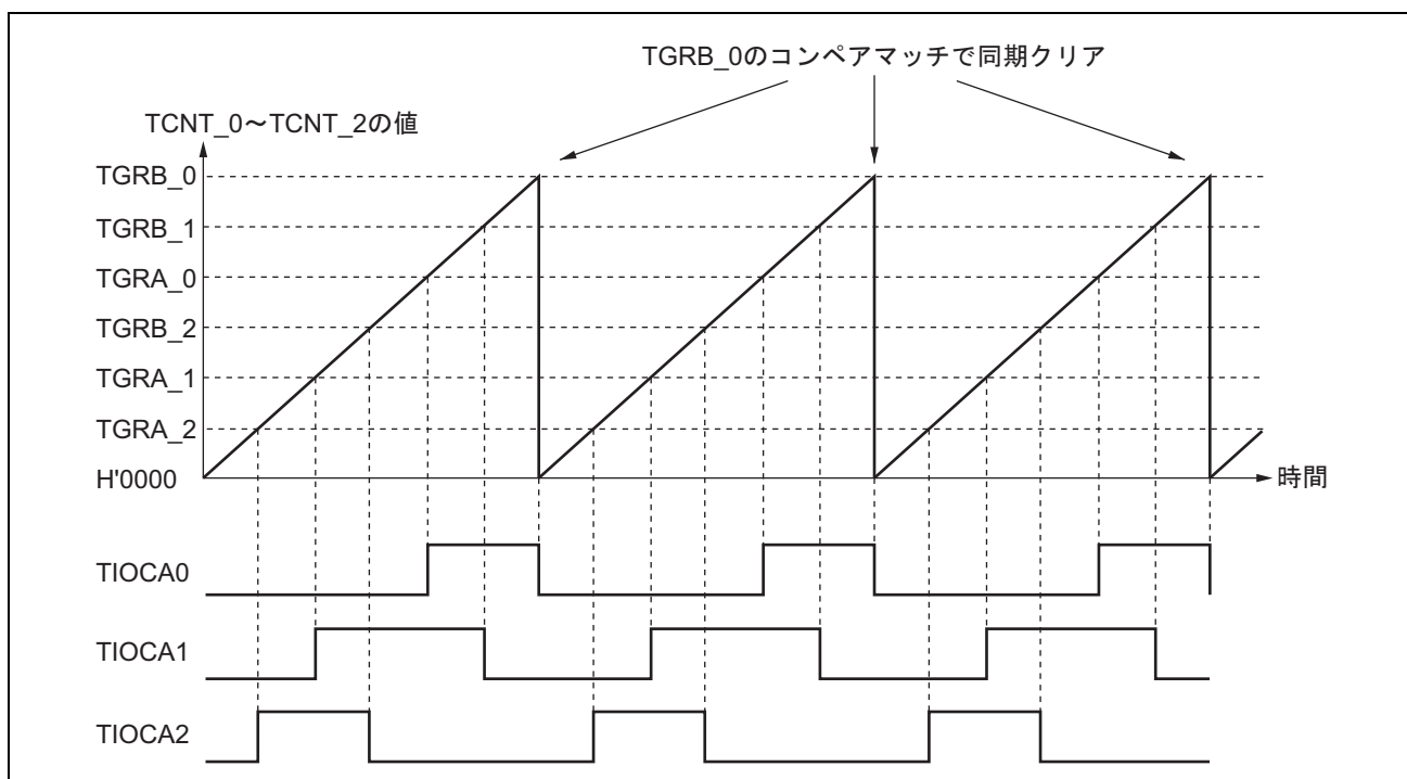
図 13.12 同期動作の動作例
