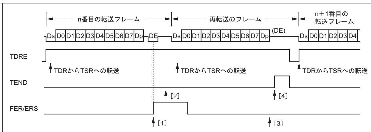
図 17.29 SCI 送信モードの場合の再転送動作
