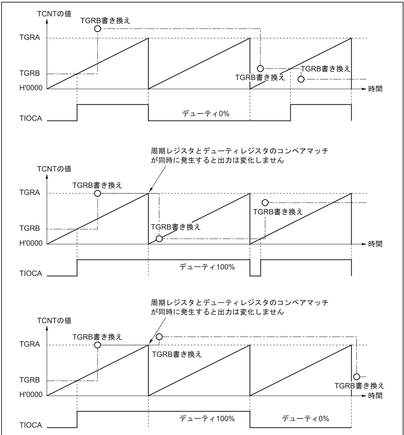
図 13.24 PWM モード動作例 (3)
