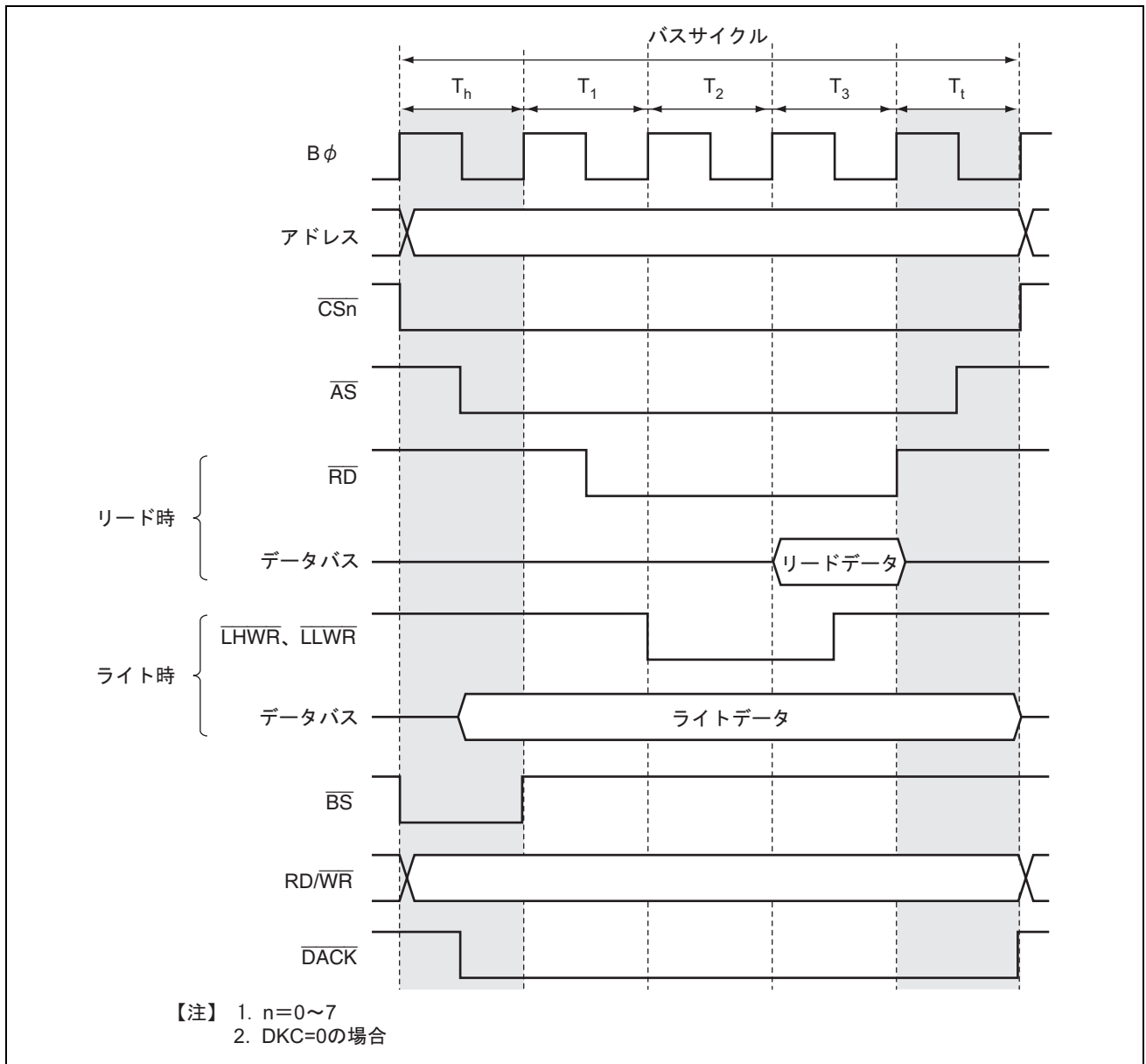
図 9.22 チップセレクトアサート期間拡張時タイミング例
