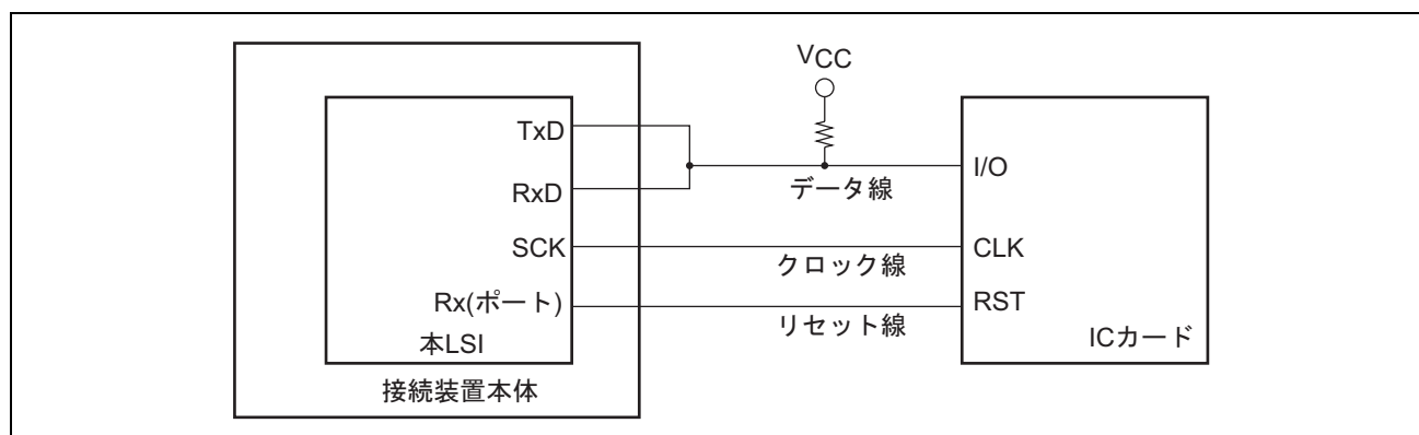
図 17.24 スマートカードインタフェース端子接続概要
