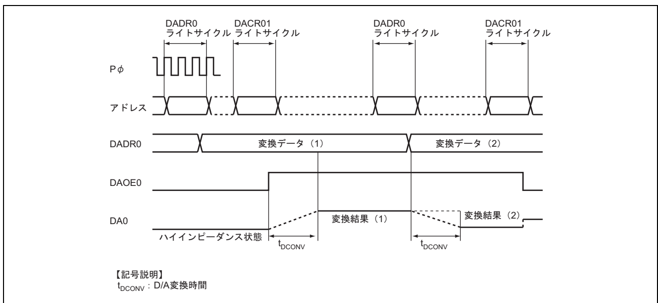
図 20.2 D/A 変換器の動作例
