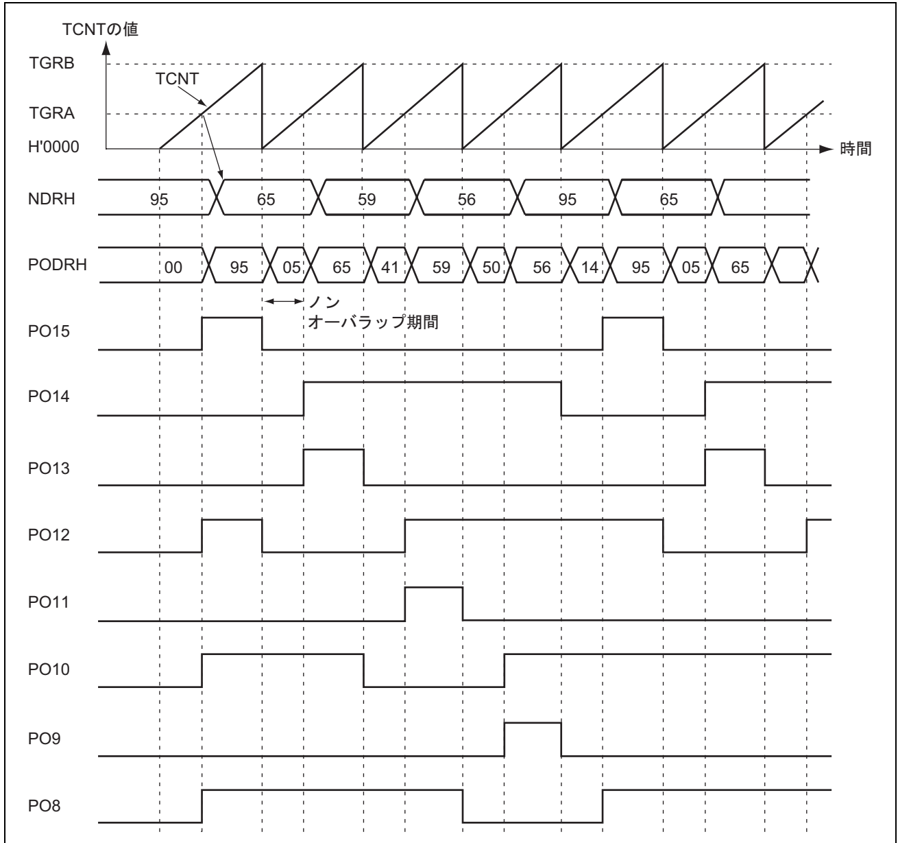
図 14.12 パルス出力ノンオーバーラップ動作例 (4相の相補ノンオーバーラップ出力)
