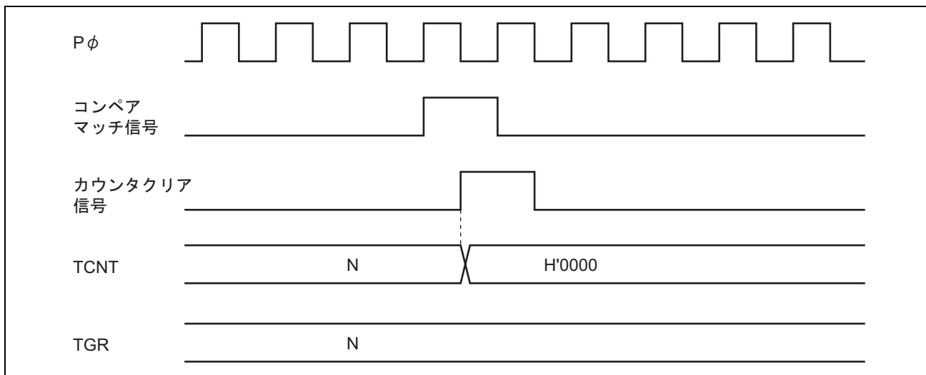
図 13.35 カウンタクリアタイミング (コンペアマッチ)
