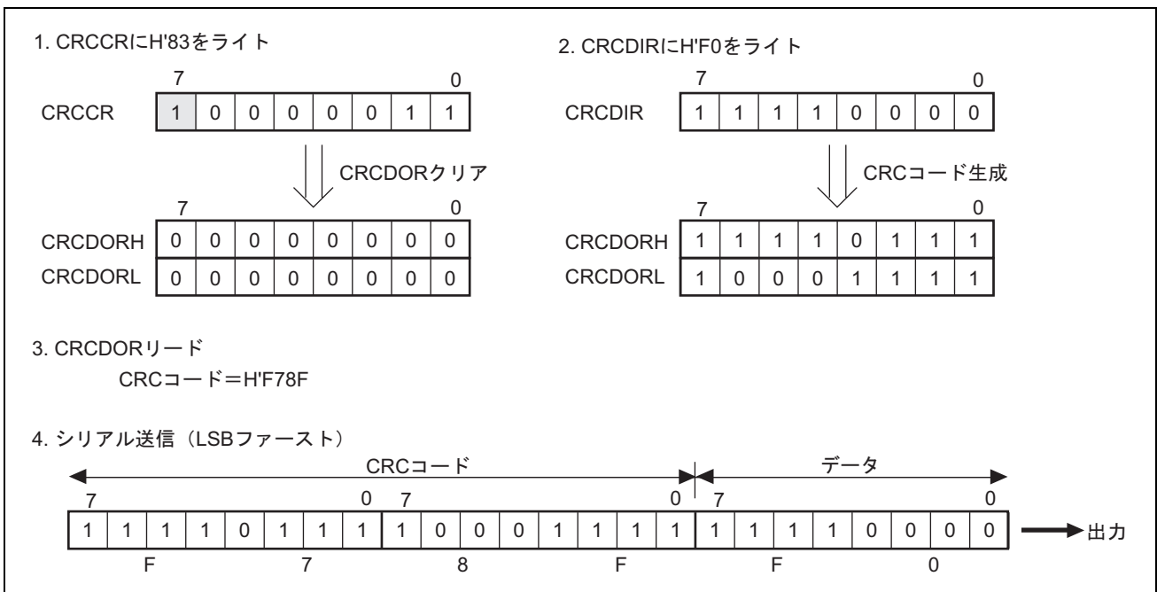
図 17.44 LSB ファーストでのデータ送信
