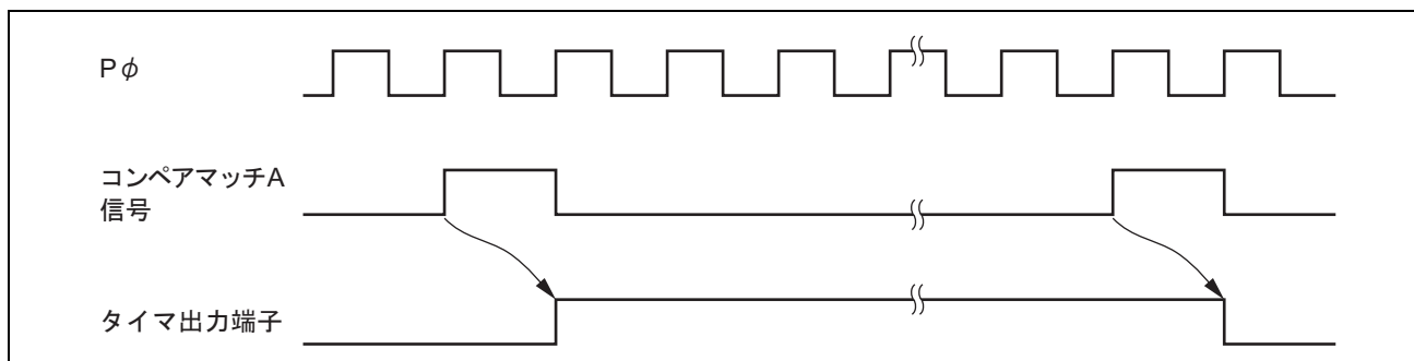
図 15.10 コンペアマッチ A 信号によるトグル出力のタイマ出力タイミング
