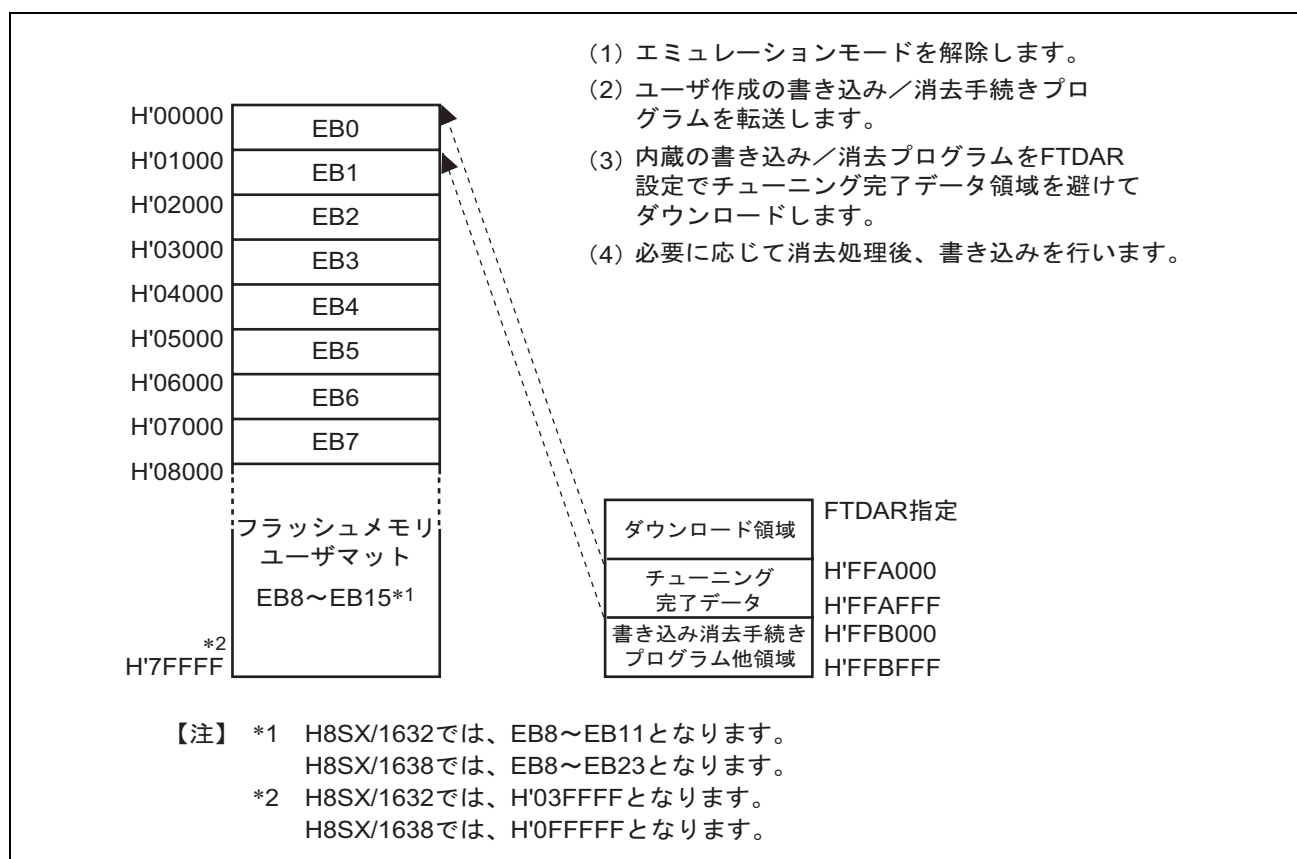
図 22.19 チューニング終了データの書き込み (H8SX/1634)
