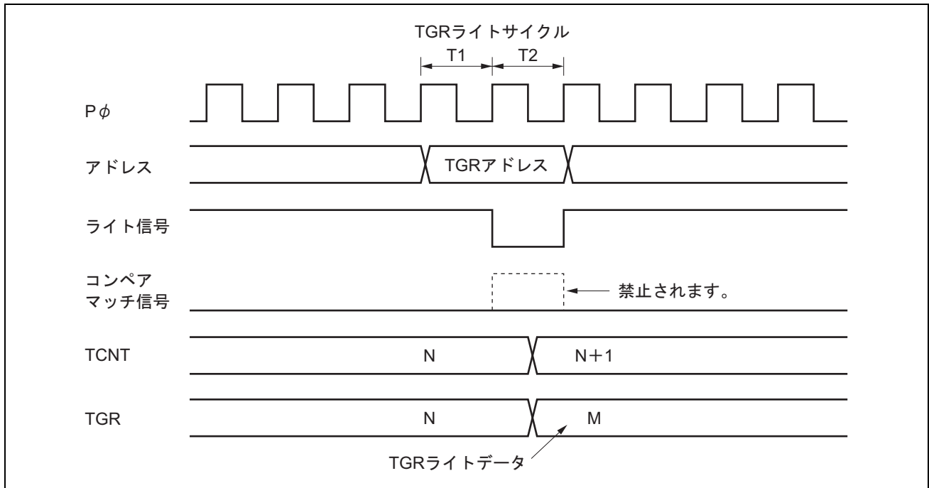
図 13.49 TGRのライトとコンペアマッチの競合
