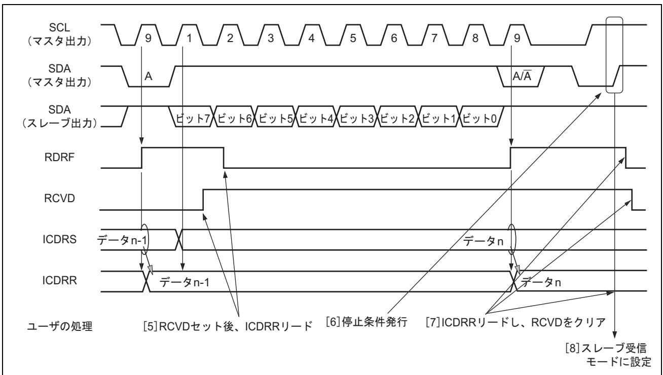
図 18.8 マスタ受信モード動作タイミング 2
