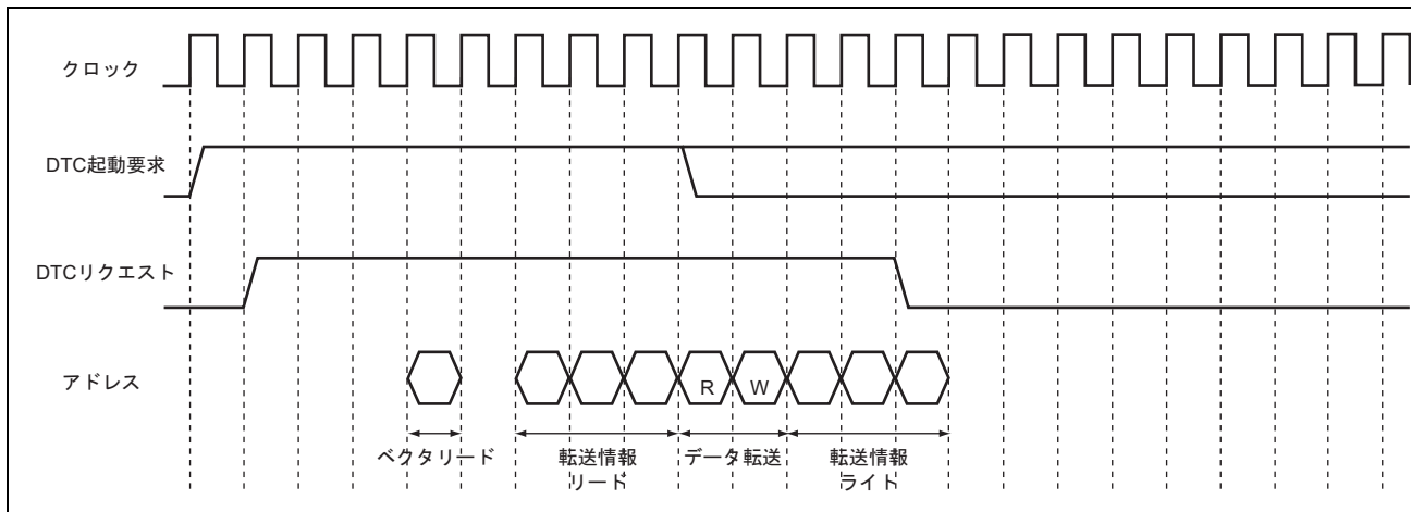
図 11.11 DTC の動作タイミング例 (ショートアドレスモード、ノーマル転送モード、リピート転送モード)
