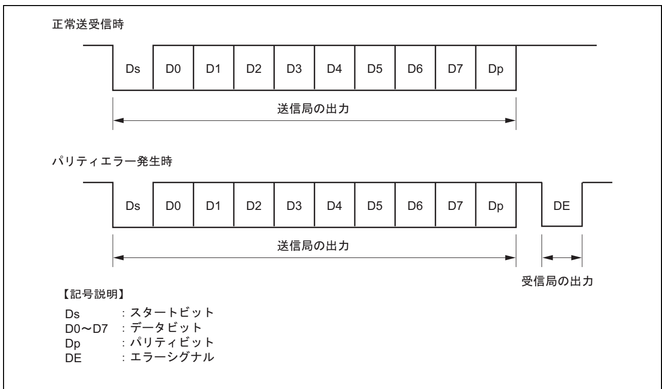
図 17.25 通常のスマートカードインタフェースのデータフォーマット
