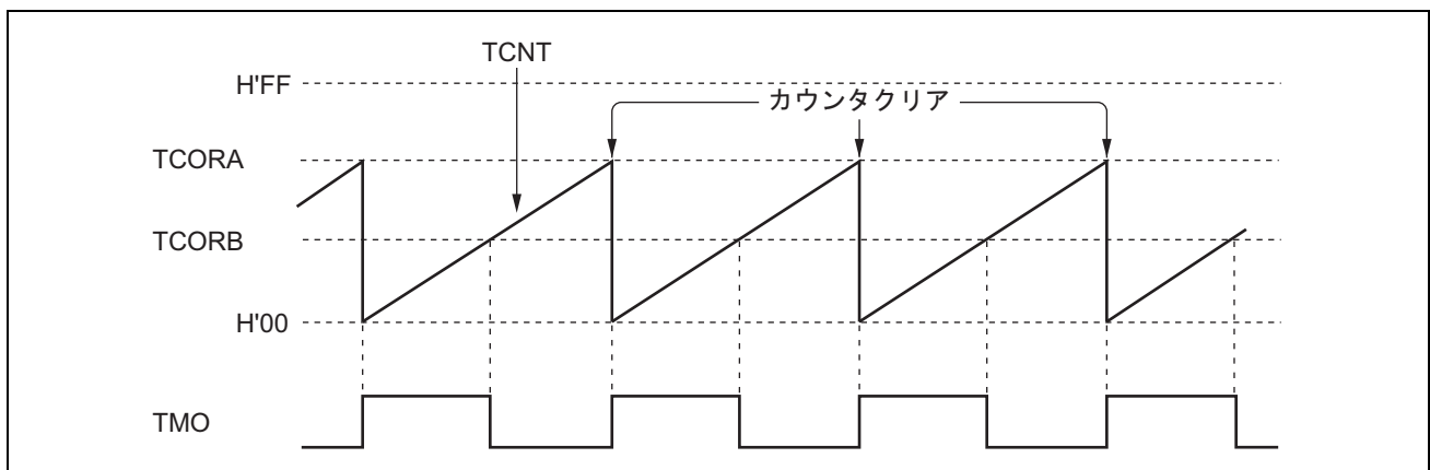
図 15.5 パルス出力例
