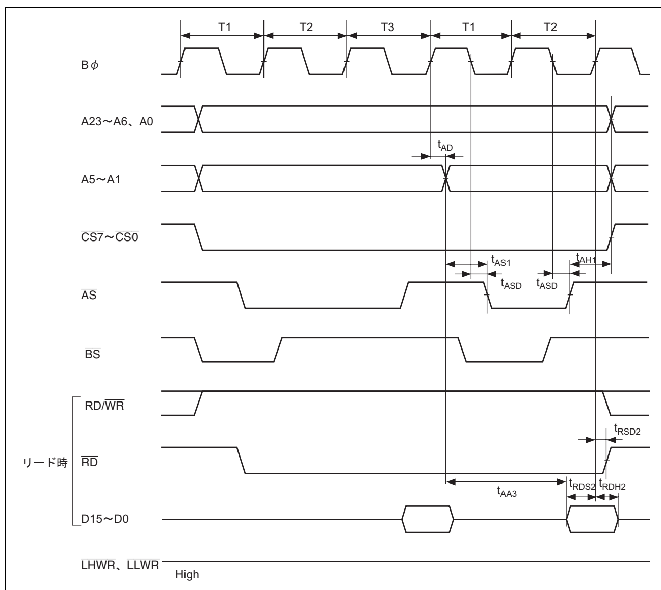
図 27.16 バースト ROM アクセスタイミング/2 ステートバーストアクセス
