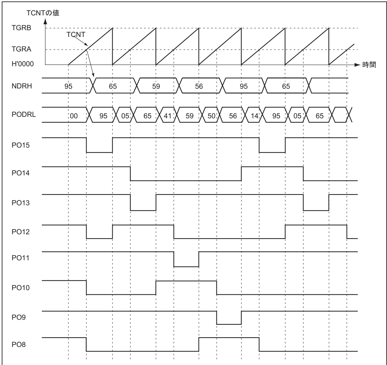
図 14.13 パルス反転出力例
