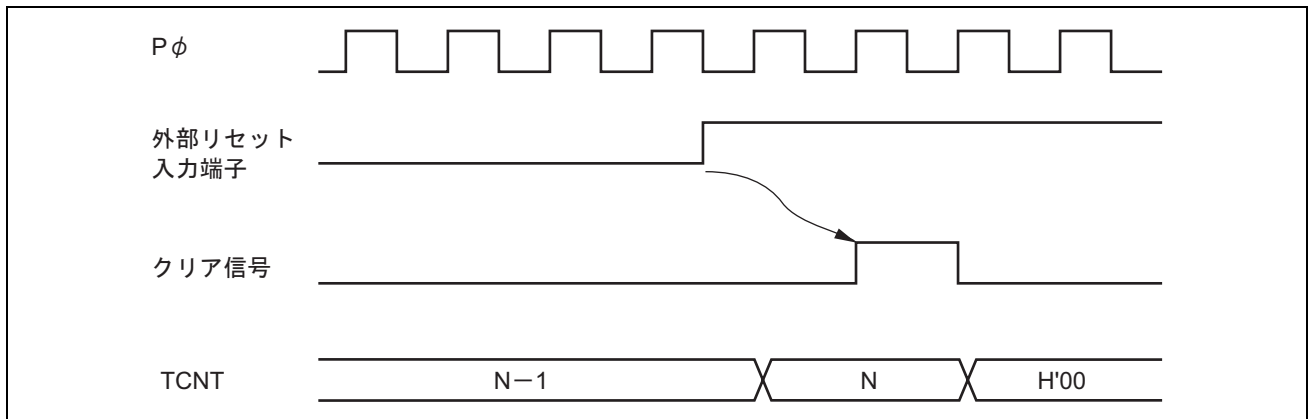
図 15.12 外部リセット入力によるクリアタイミング (立ち上がりエッジ)
