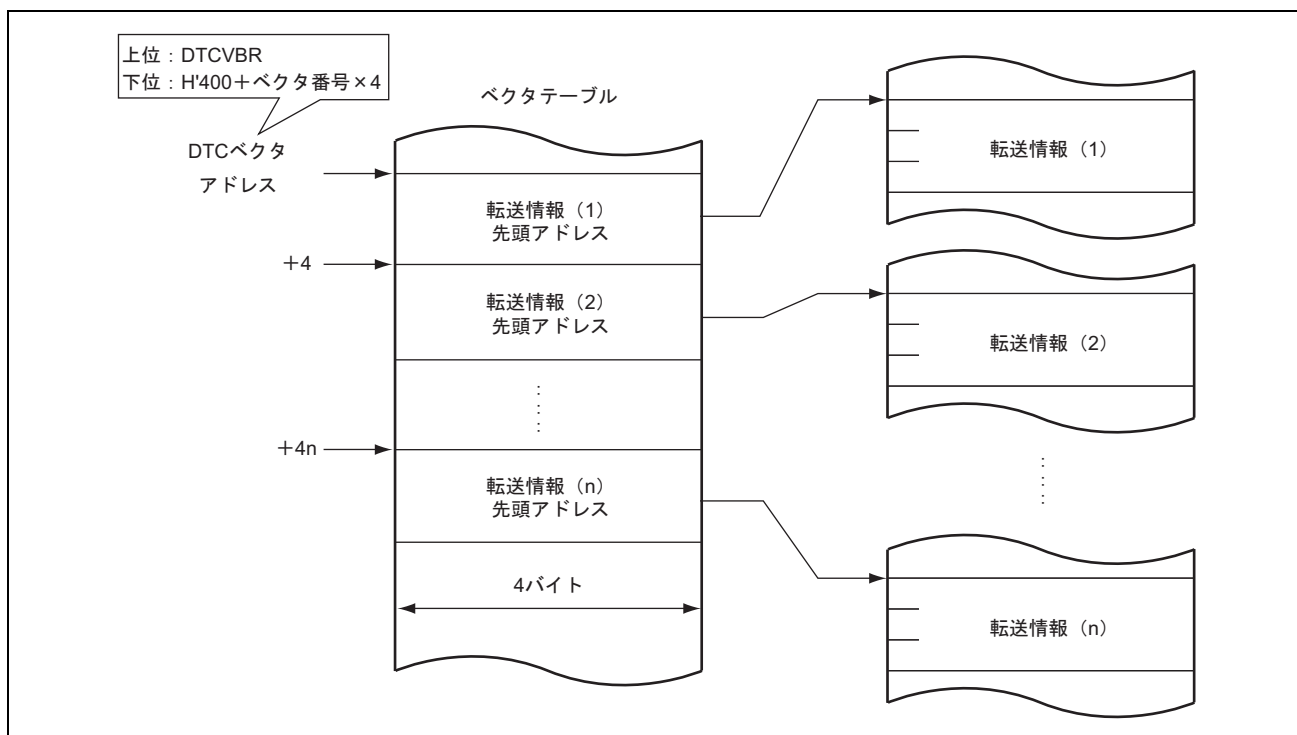
図 11.3 DTC ベクタテーブルと転送情報の対応
