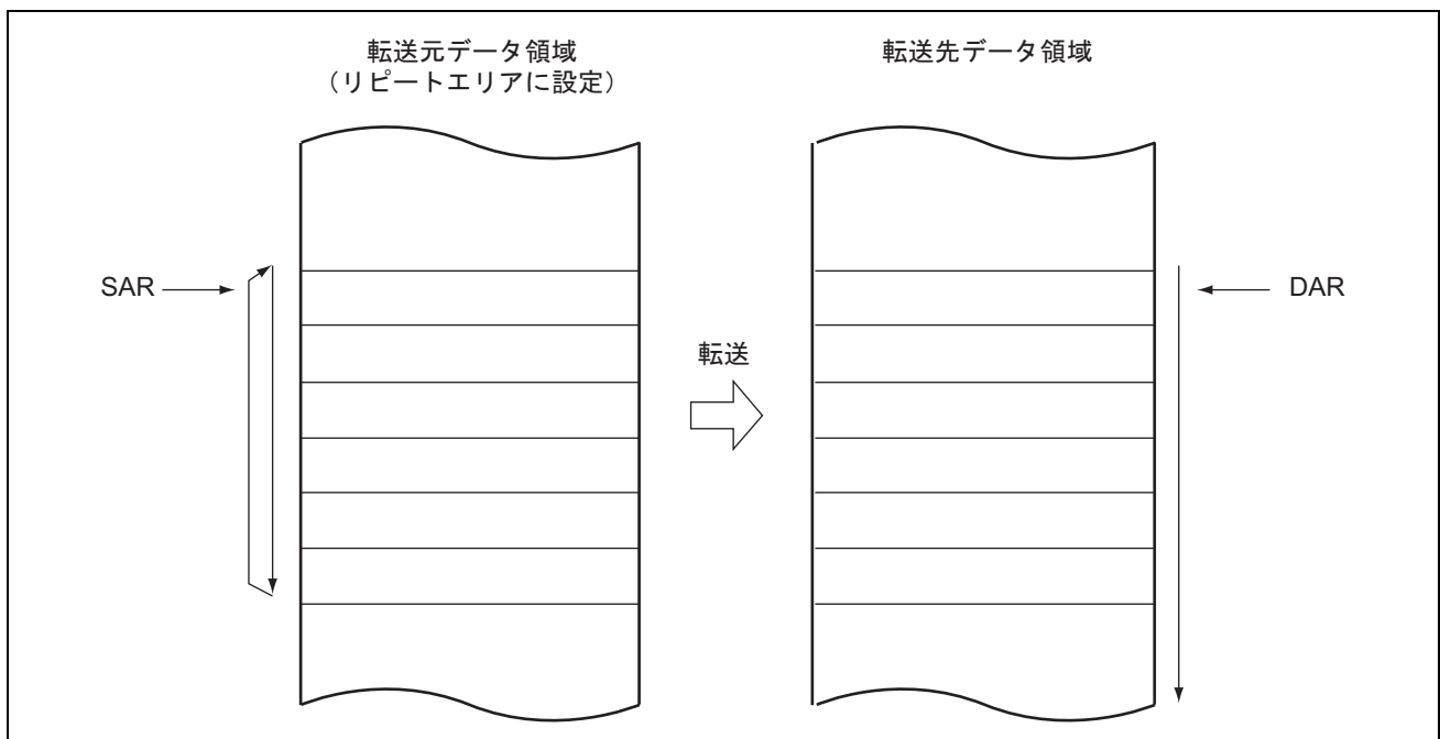
図 11.8 リピート転送モードのメモリマップ (転送元をリピートエリアに指定した場合)
