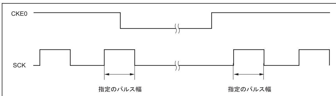
図 17.34 クロック出力固定タイミング
