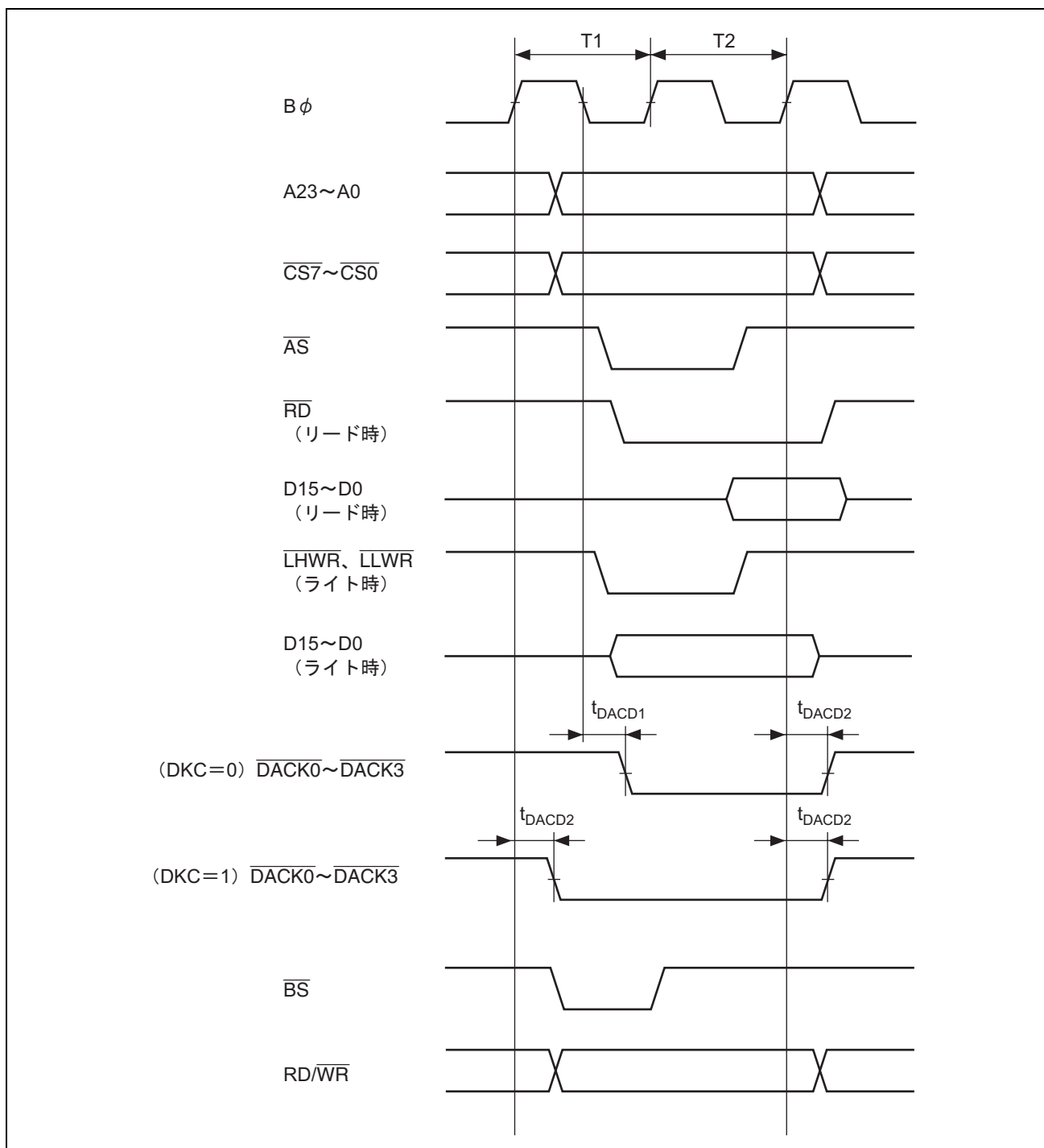
図 27.23 DMAC シングルアドレス転送タイミング (2 ステートアクセス)
