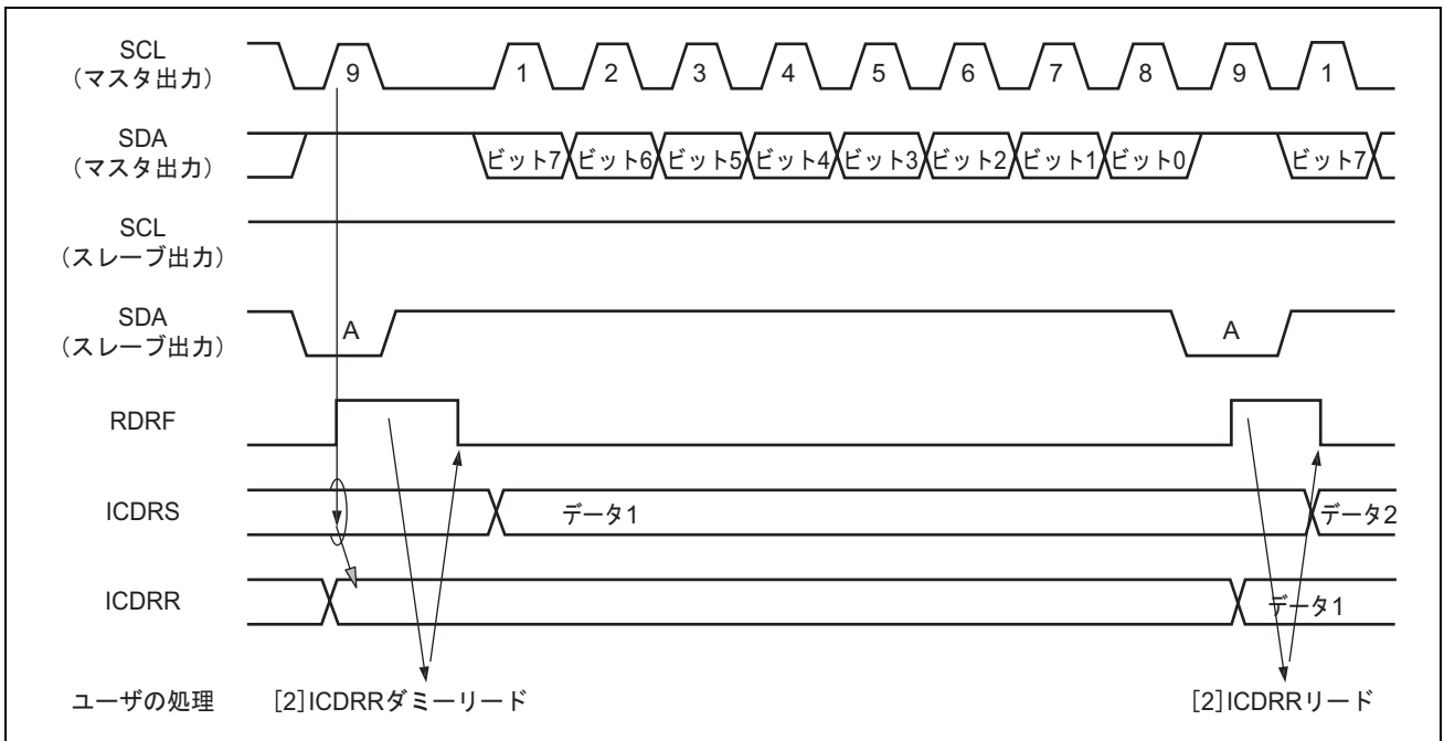
図 18.11 スレーブ受信モード動作タイミング 1
