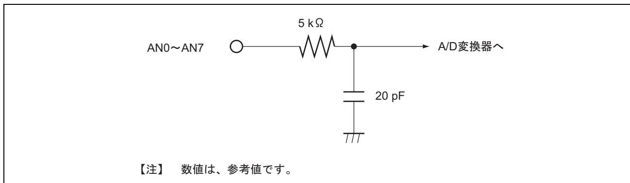
図 19.14 アナログ入力端子等価回路
