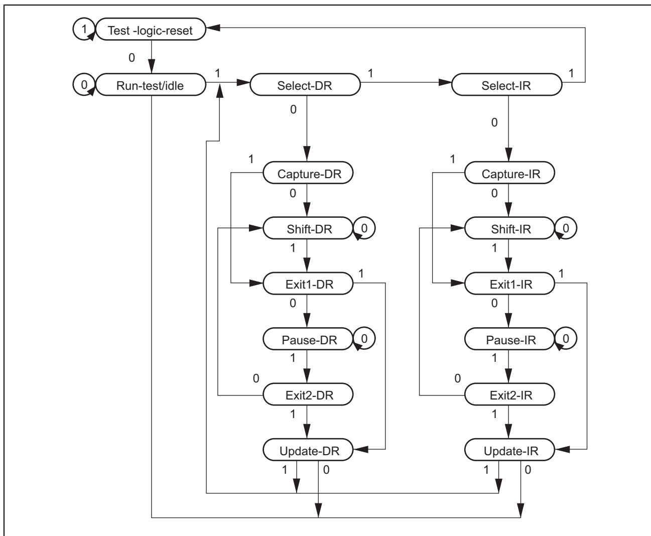
図 23.2 TAP コントローラ
