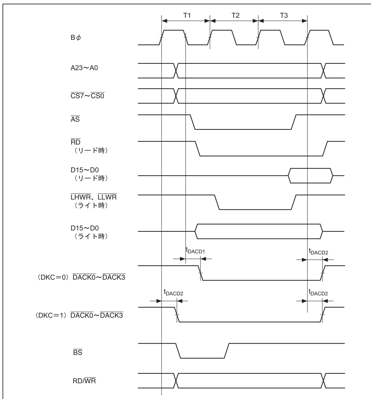
図 27.24 DMAC シングルアドレス転送タイミング (3 ステートアクセス)
