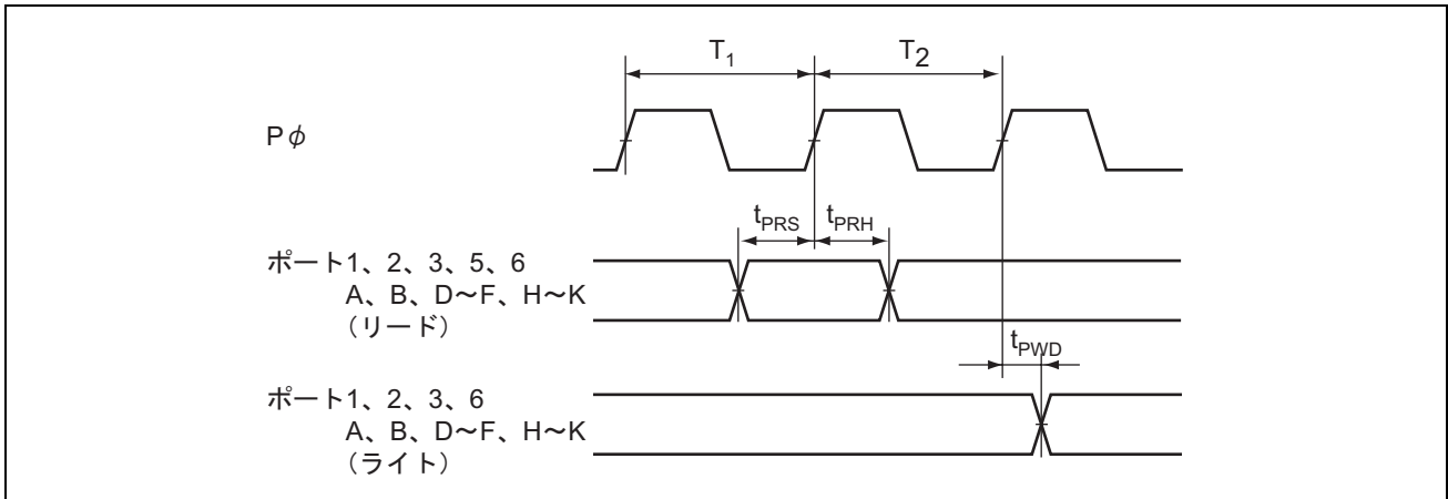
図 27.25 I/O ポート入出力タイミング
