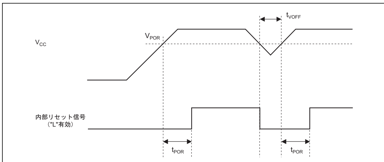
図 27.40 パワーオンリセットタイミング
