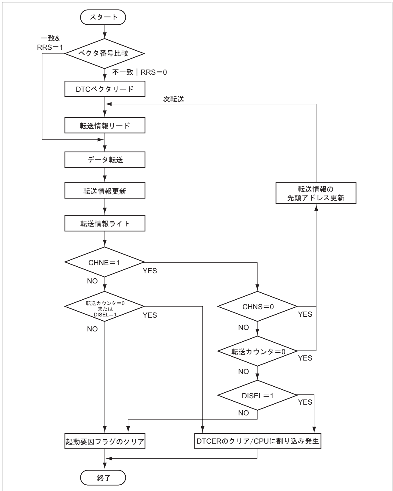
図 11.4 DTC 動作フローチャート
