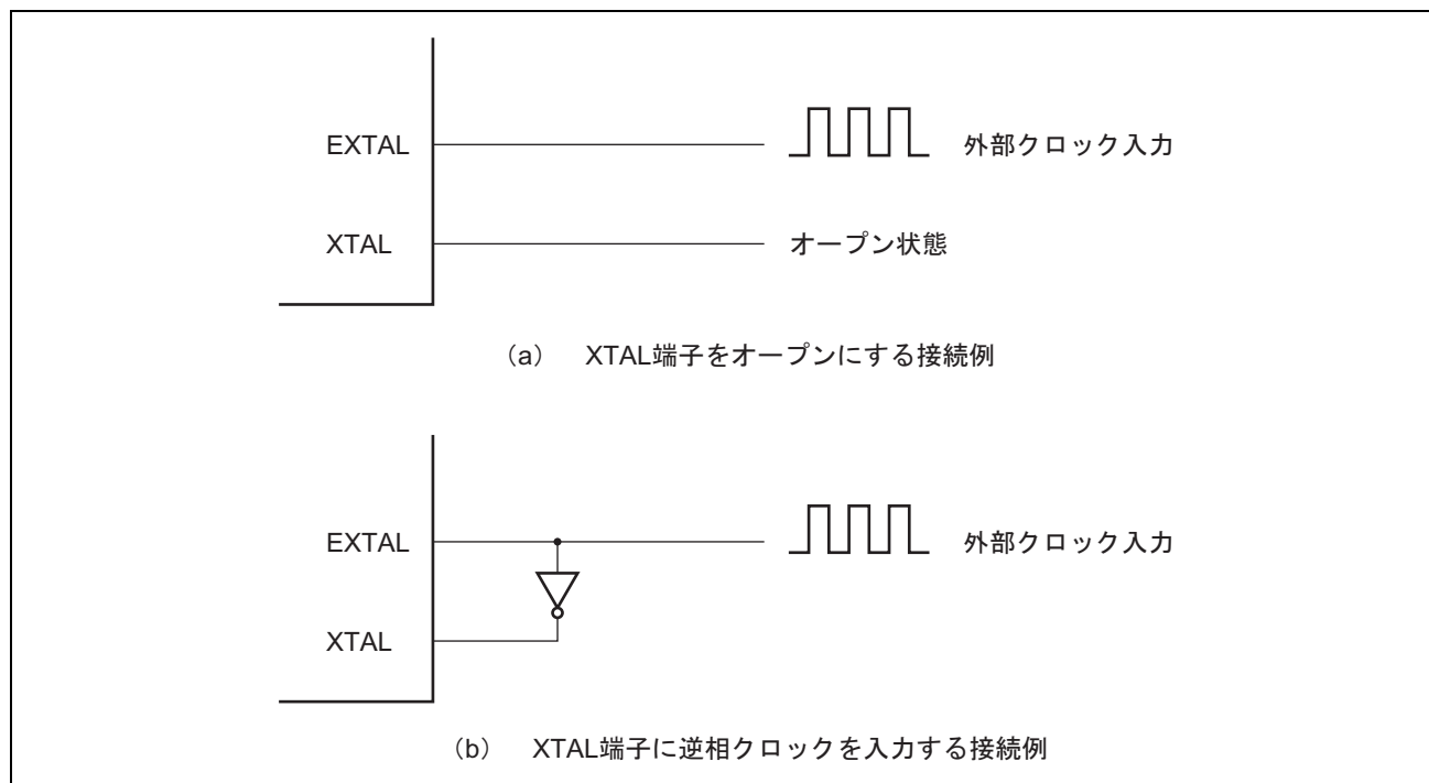
図 24.4 外部クロックの接続例
