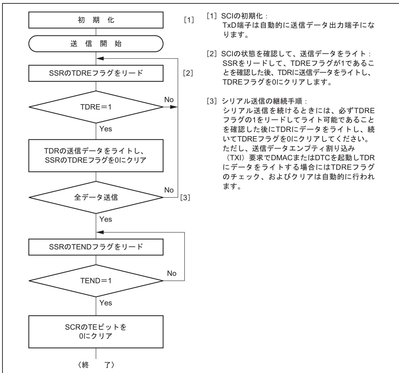
図 17.20 シリアル送信のフローチャートの例
