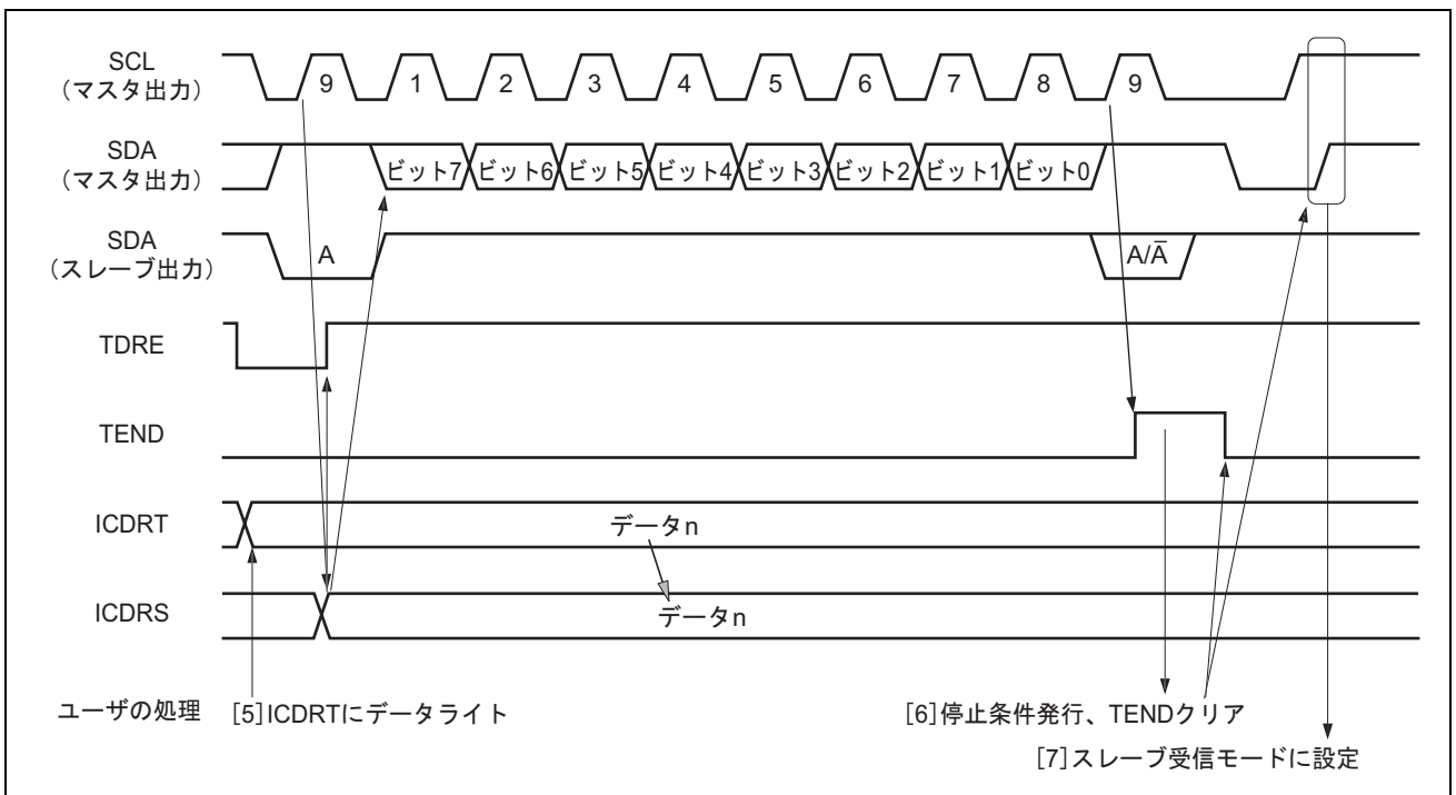
図 18.6 マスタ送信モード動作タイミング 2
