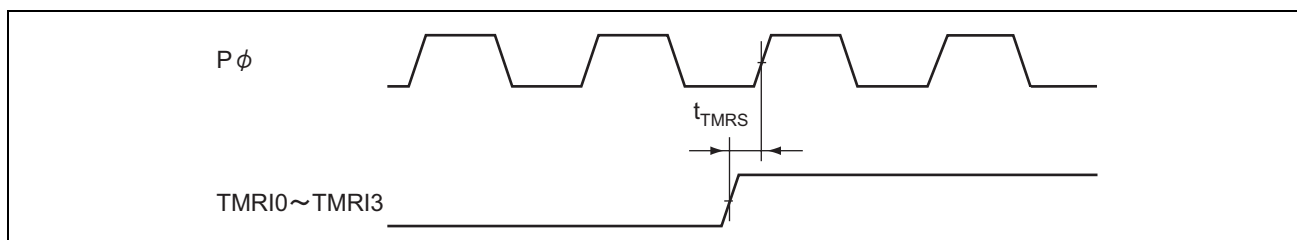
図 27.30 8ビットタイマリセット入力タイミング
