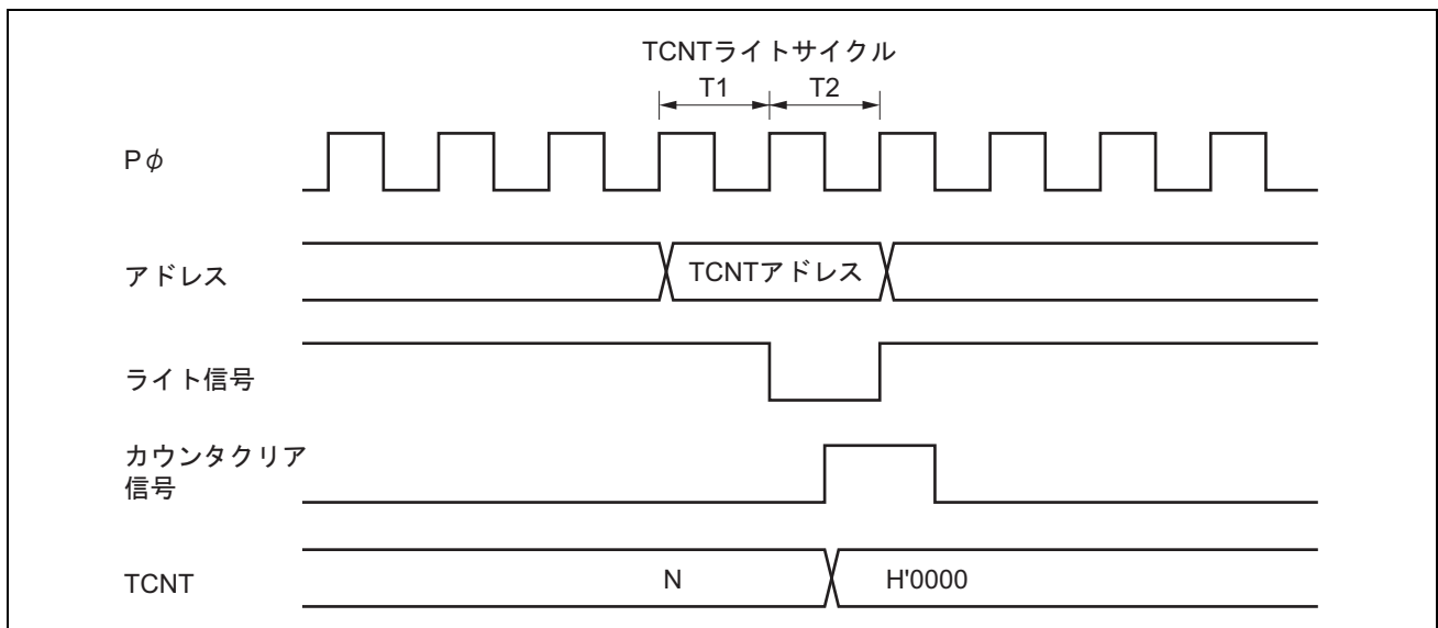
図 13.47 TCNTのライトとクリアの競合
