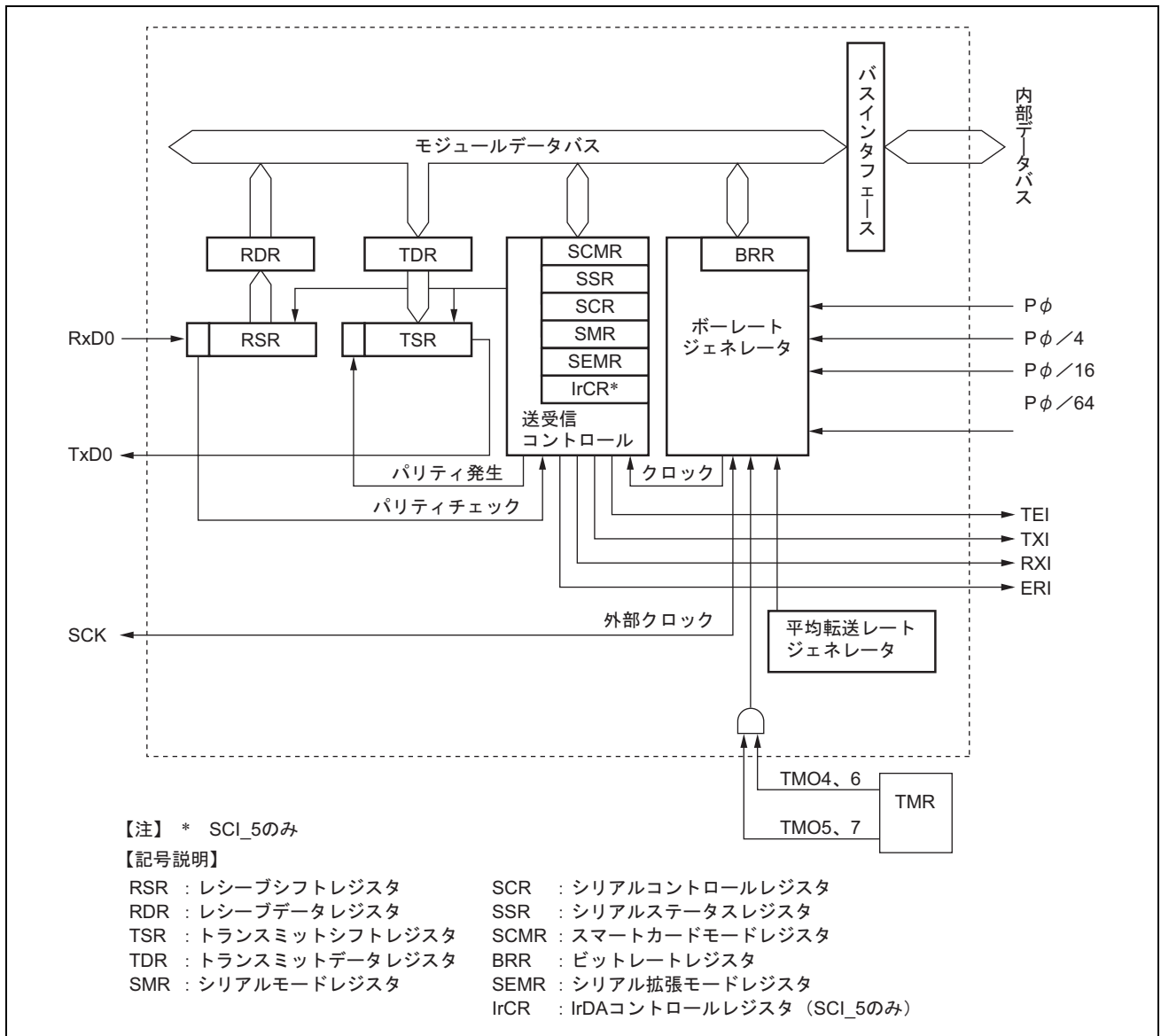
図 17.2 SCI_5、6 のブロック図
