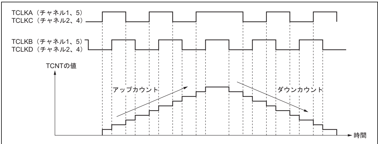
図 13.26 位相計数モード 1 の動作例
