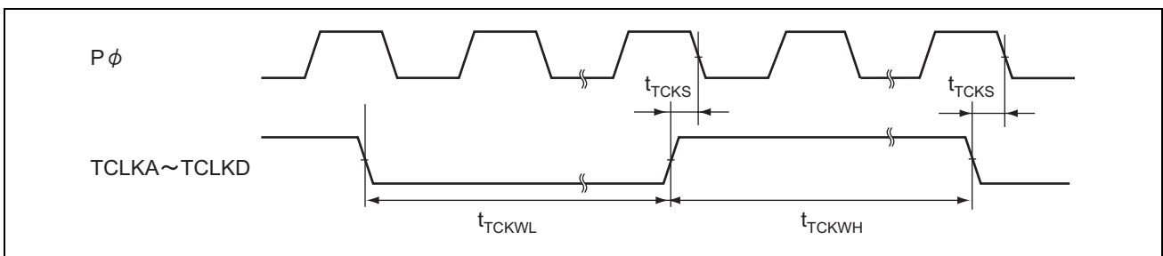
図 27.27 TPU クロック入力タイミング
