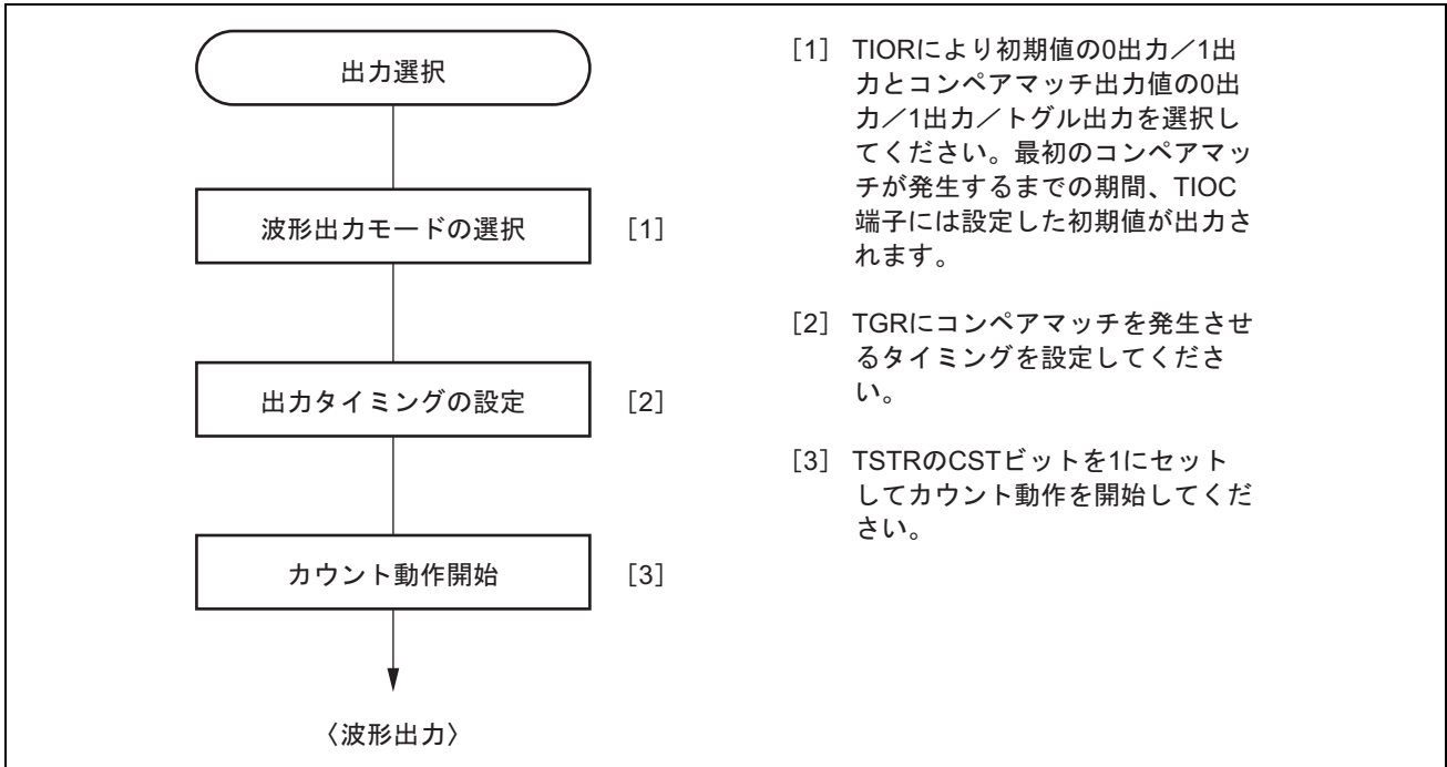
図 13.6 コンペアマッチによる波形出力動作例
