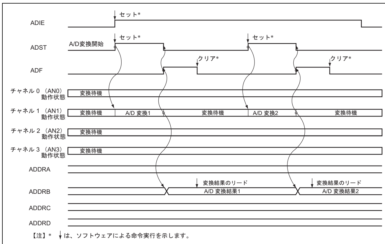
図 19.3 A/D 変換器の動作例（シングルモード、チャンネル 1 選択時）
