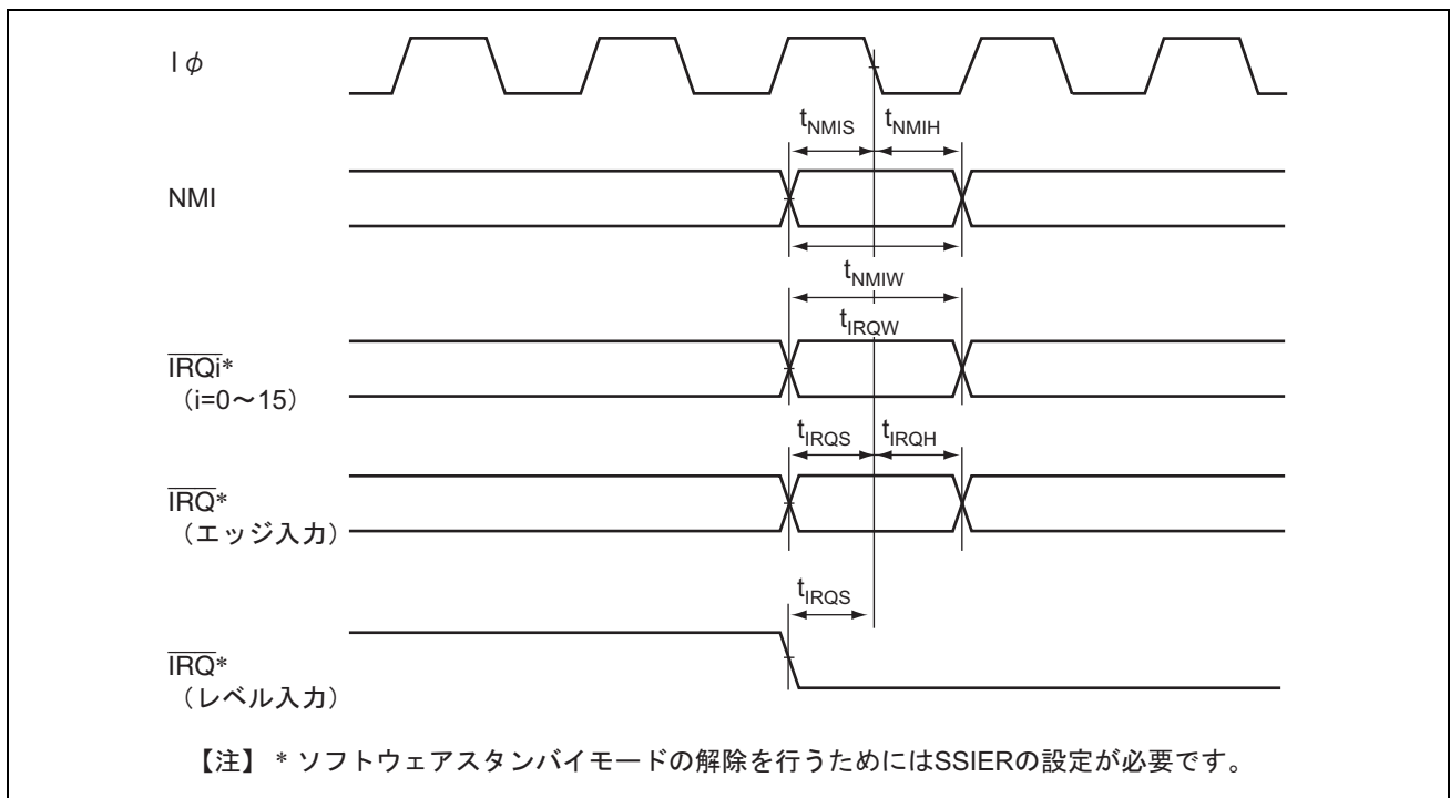
図 27.7 割り込み入力タイミング
