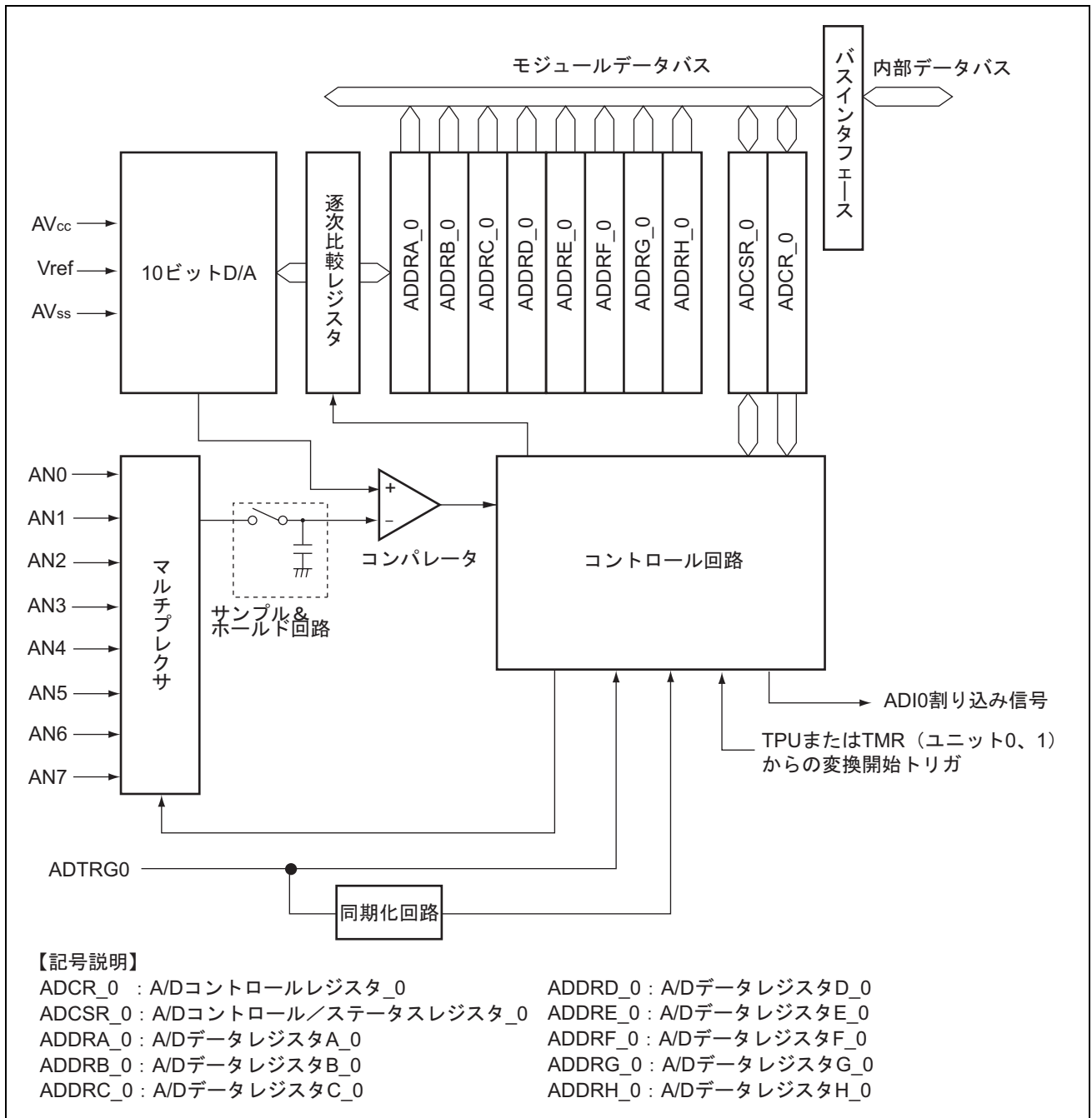
図 19.1 A/D 変換器 (ユニット0/AD_0) のブロック図
