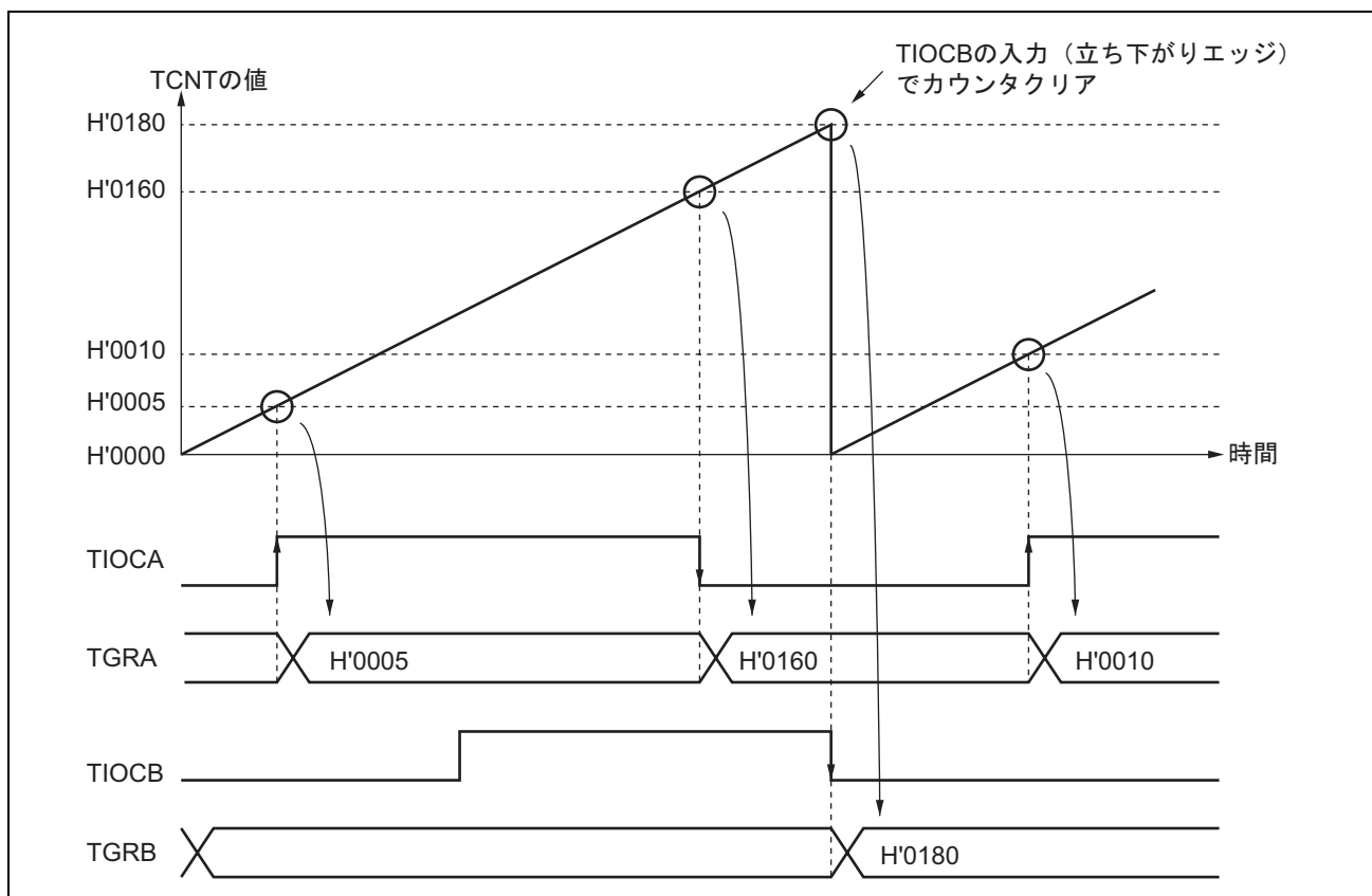
図 13.10 インพุットキャプチャ動作例
