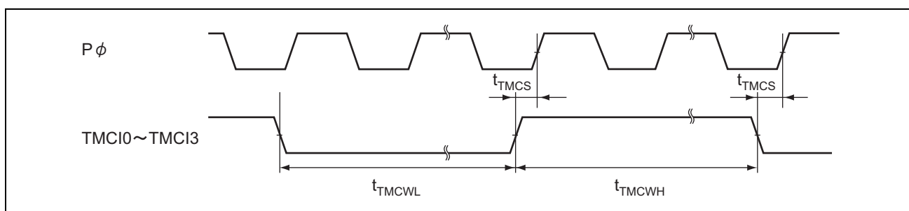
図 27.31 8ビットタイマクロック入力タイミング
