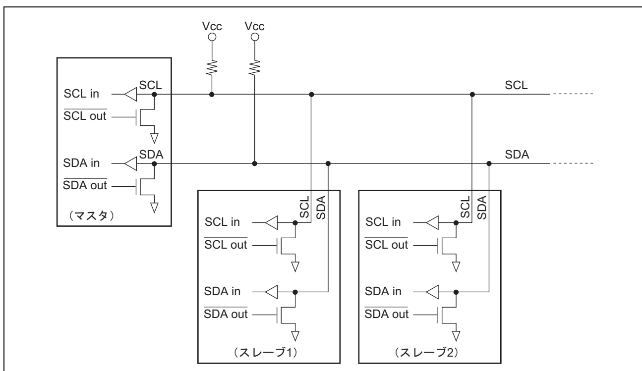
図 18.2 入出力端子の外部回路接続例
