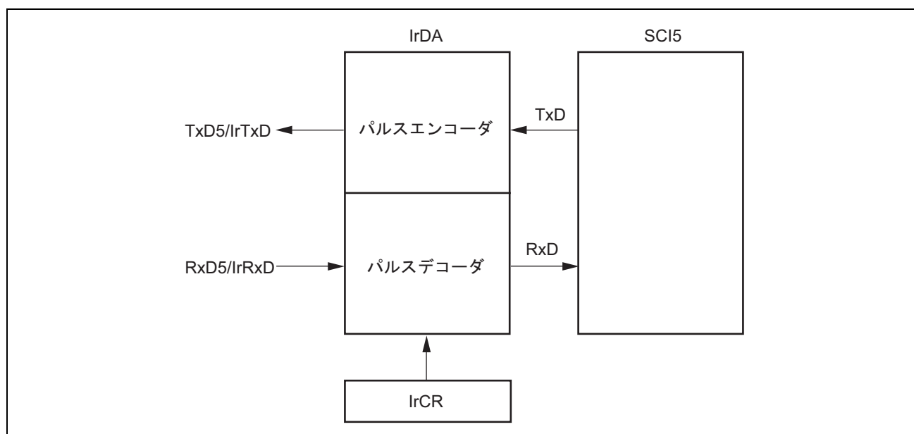
図 17.36 IrDA ブロック図
