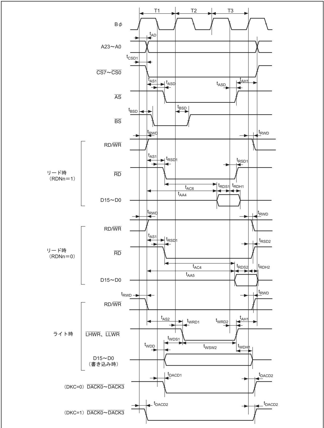
図 27.9 基本バスタイミング/3 ステートアクセス
