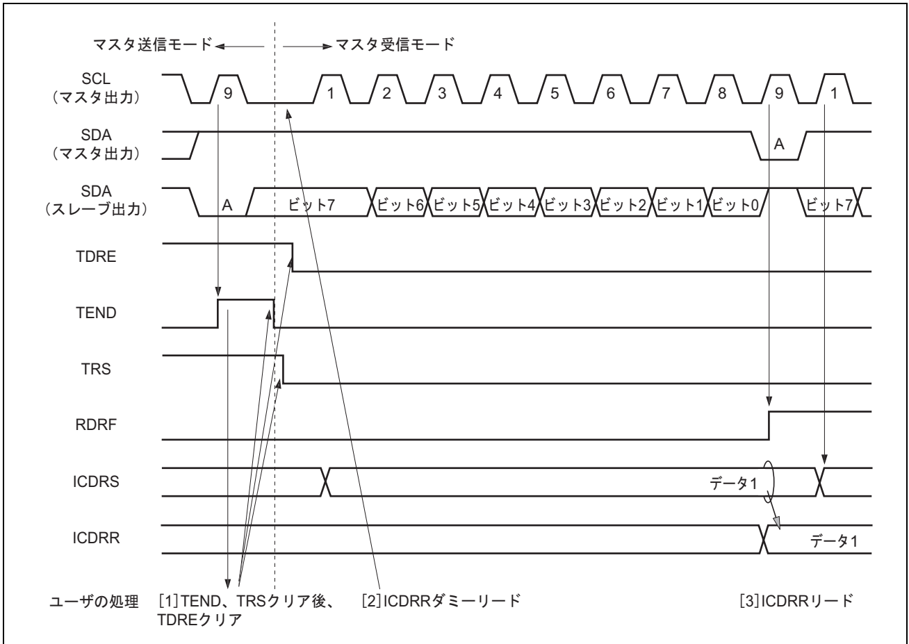
図 18.7 マスタ受信モード動作タイミング 1
