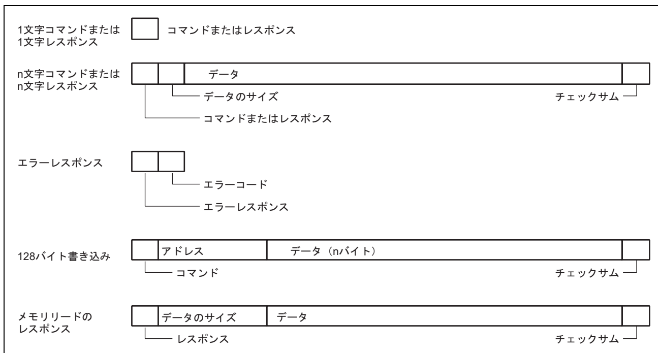
図 22.23 通信プロトコルフォーマット
