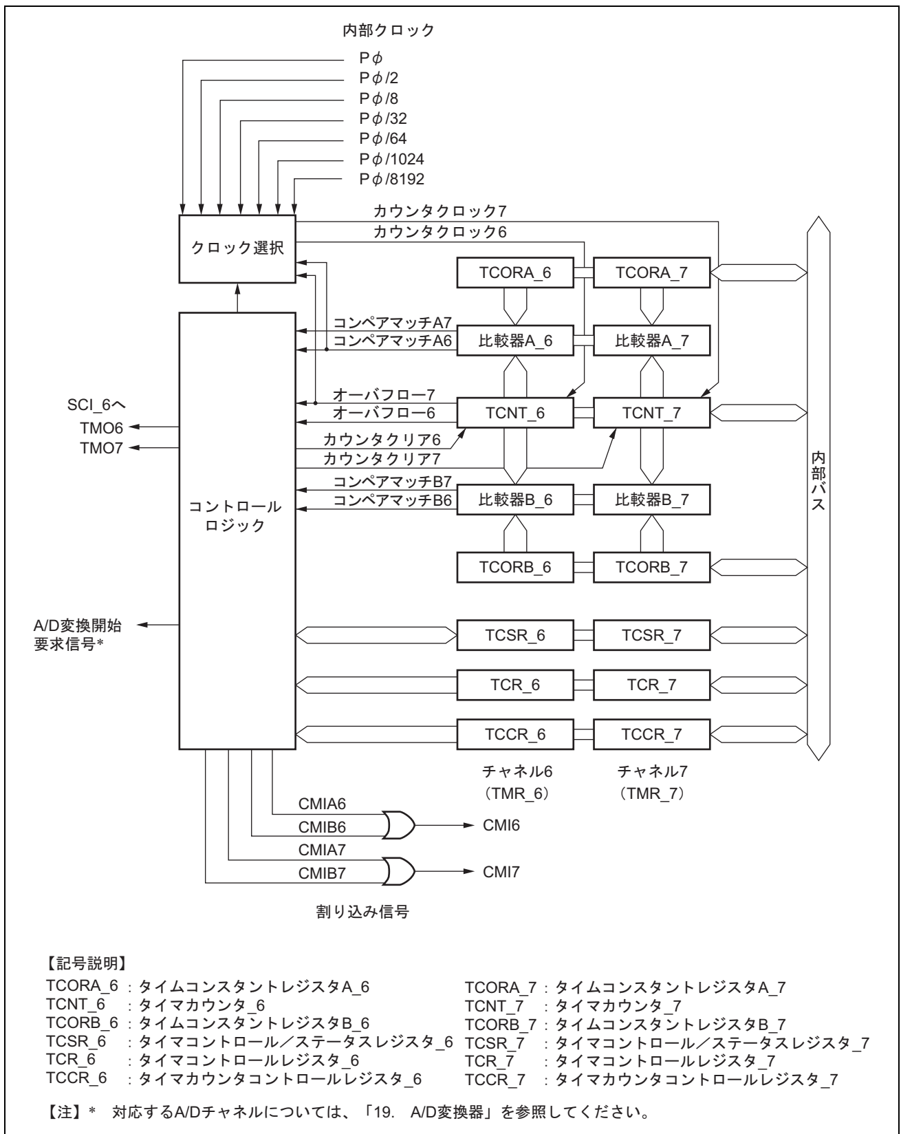
図 15.4 8ビットタイマ (ユニット3) のブロック図
