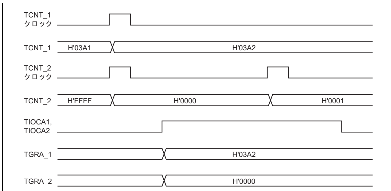
図 13.19 カスケード接続動作例 (1)
