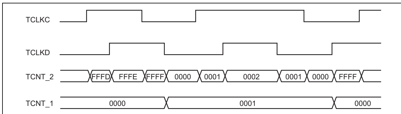
図 13.20 カスケード接続動作例 (2)
