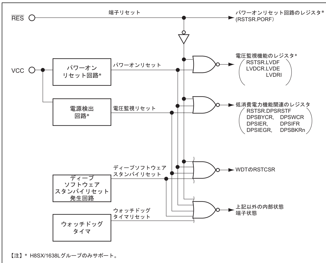
図 4.1 リセット回路のブロック図
