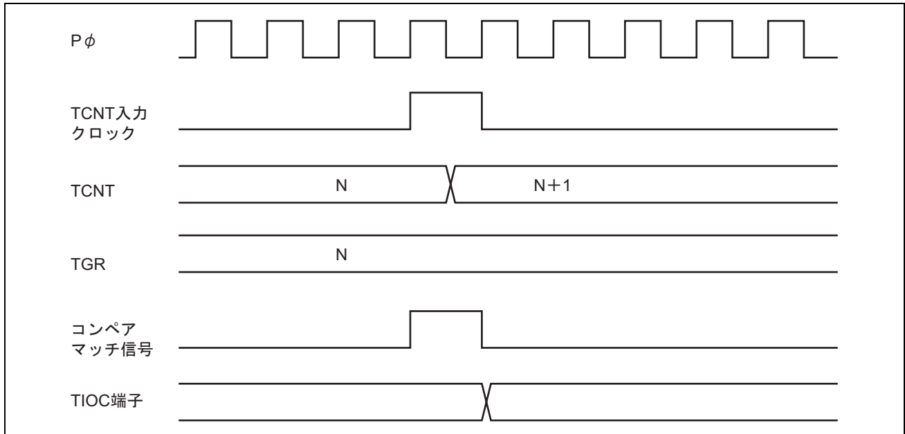
図 13.33 アウトプットコンペア出力タイミング
