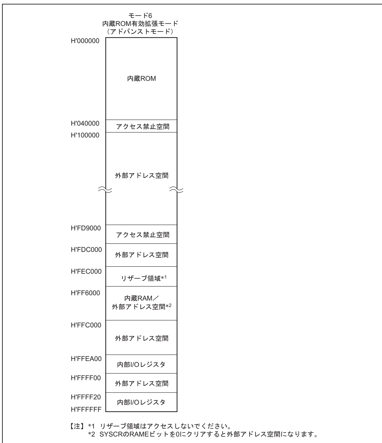
図 3.3 H8SX/1632、1632L の各動作モードのアドレスマップ (2)
