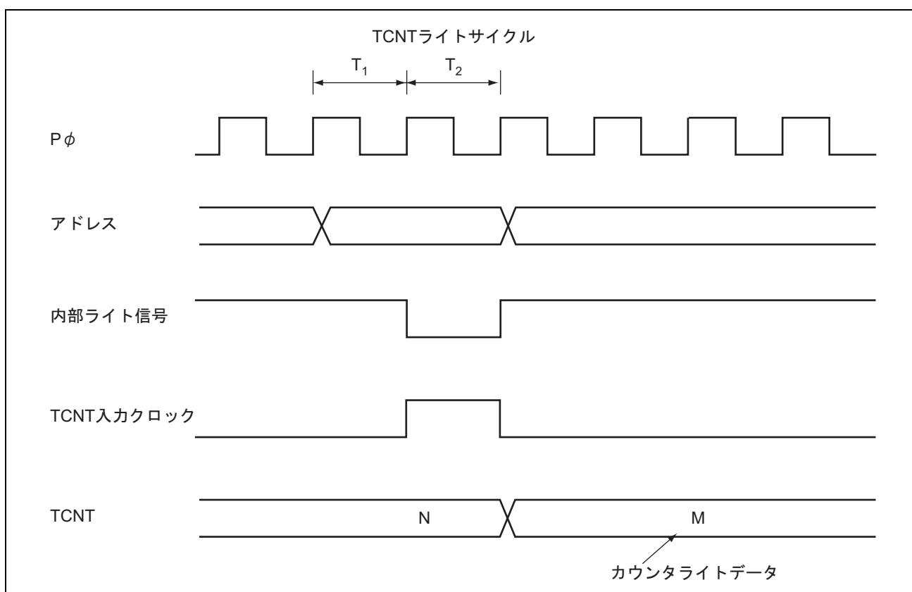
図 16.5 TCNT のライトとカウントアップの競合
