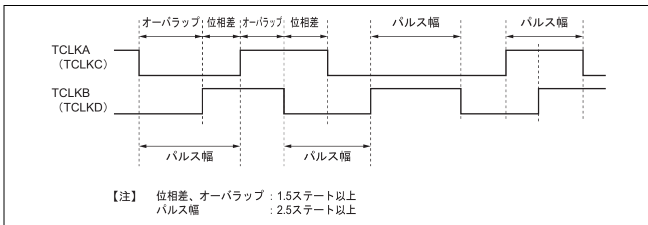
図 13.46 位相計数モード時の位相差、オーバーラップ、およびパルス幅
