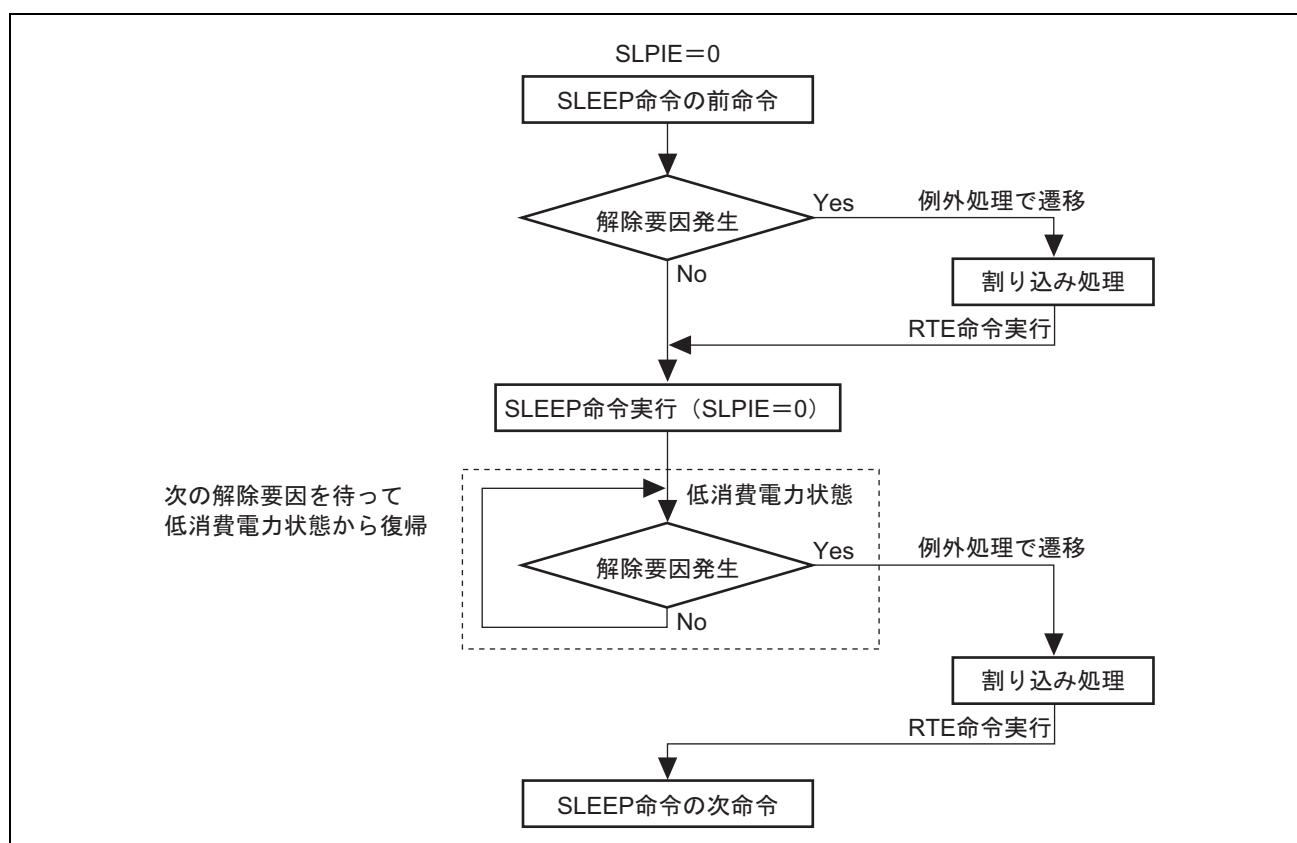
図 25.11 SLEEP 命令実行直前に解除要因割り込みが発生した場合 (スリープ命令例外処理が発生しない場合)
