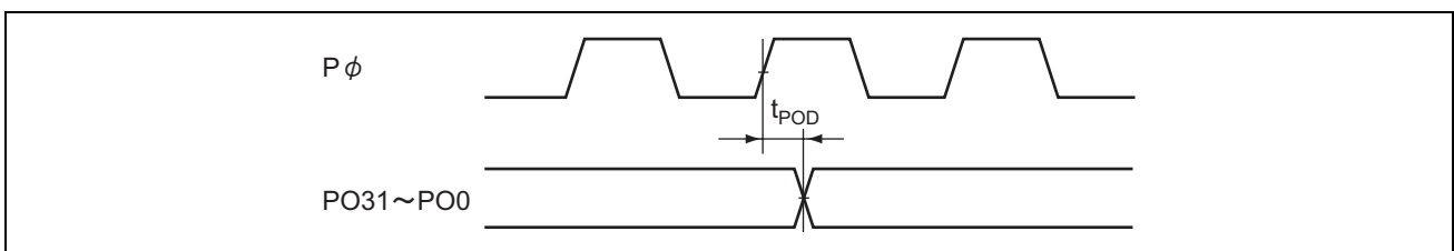
図 27.28 PPG 出力タイミング
