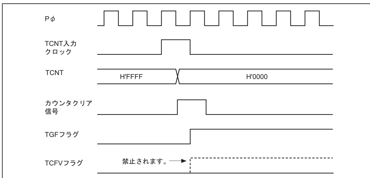
図 13.54 オーバフローとカウンタクリアの競合
