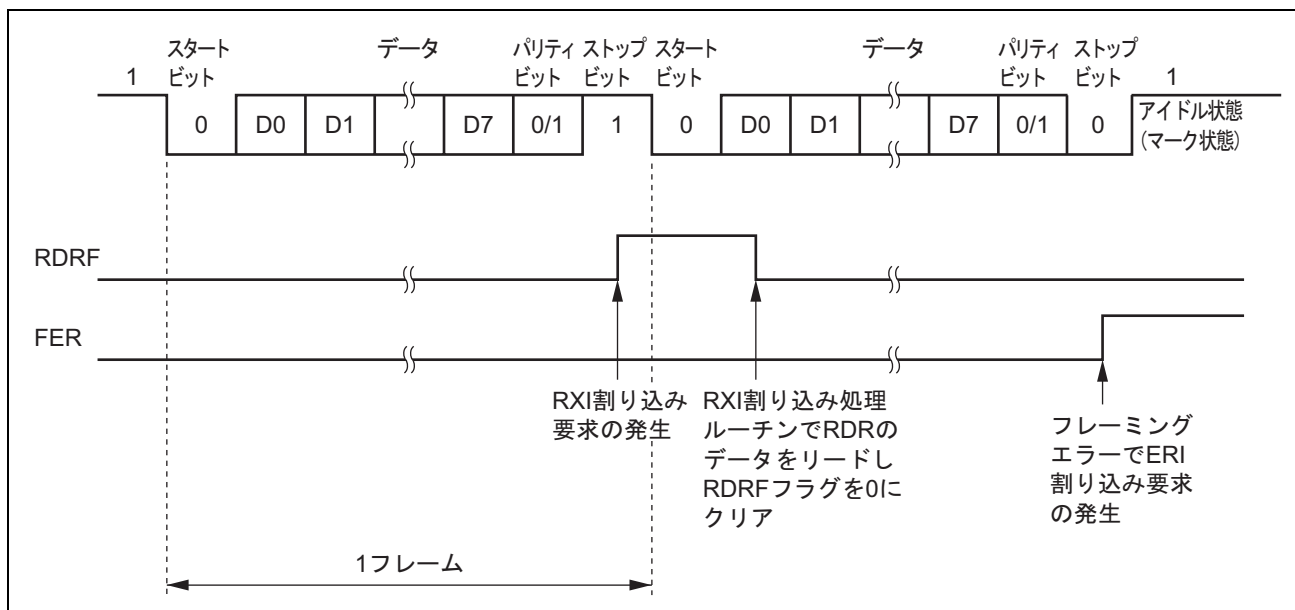
図 17.11 SCI の受信時の動作例 (8 ビットデータ/パリティあり/1 ストップビットの例)
