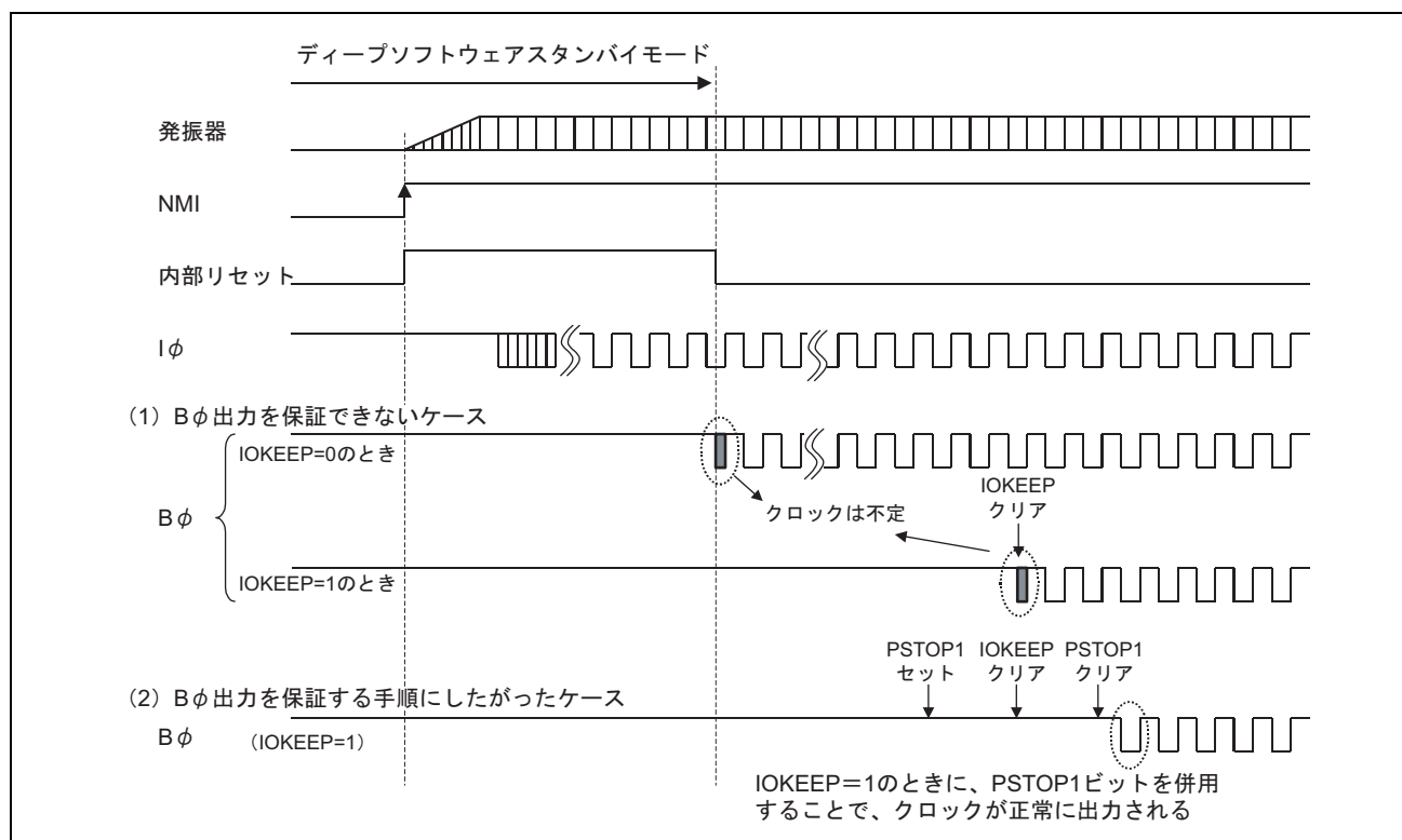
図 25.3 ディープソフトウェアスタンバイモード解除時の B \phi
