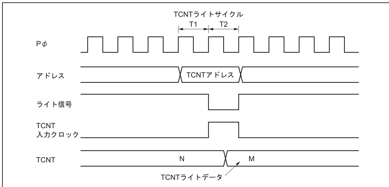
図 13.48 TCNTのライトとカウントアップの競合
