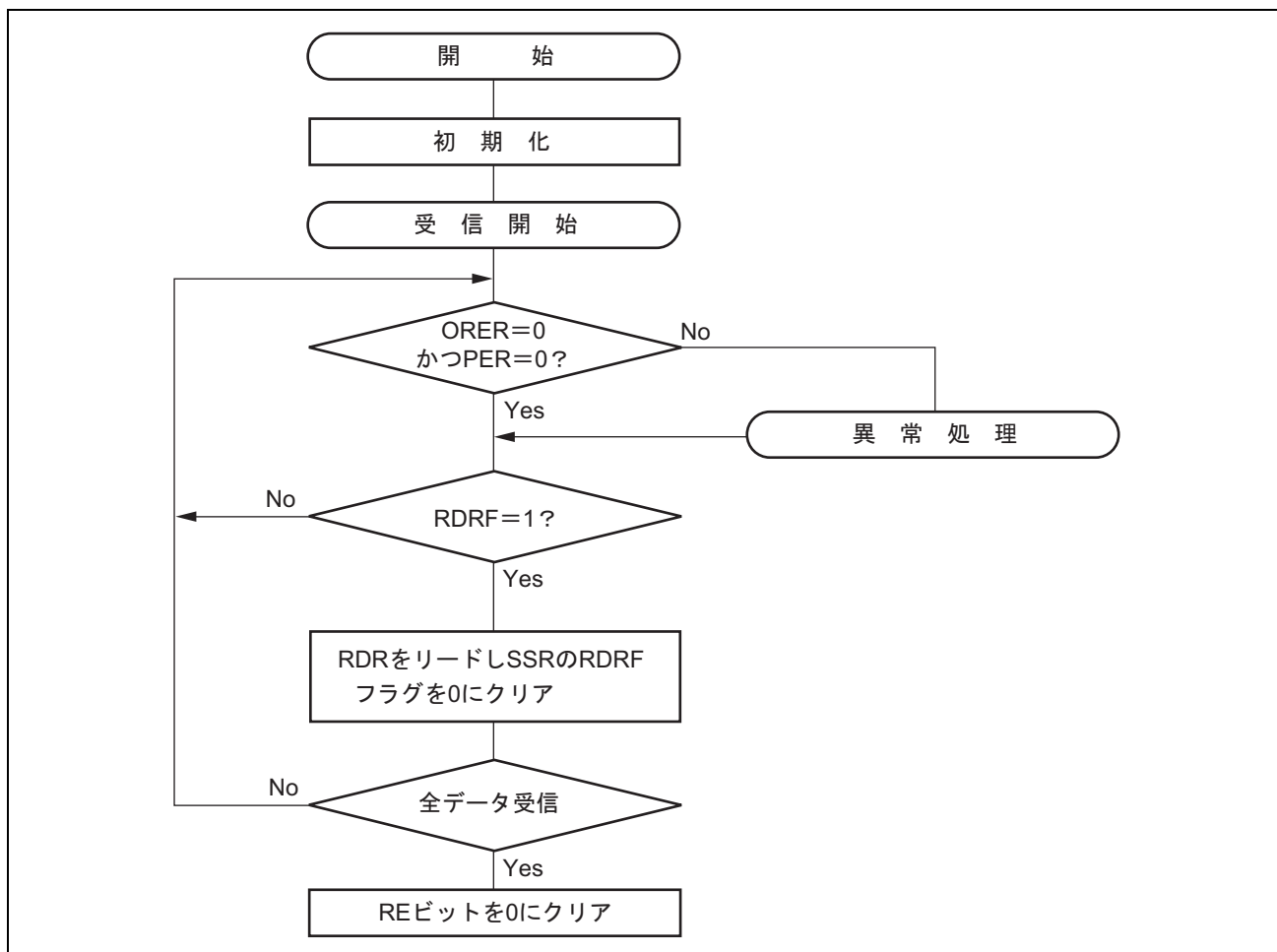
図 17.33 受信フローの例
