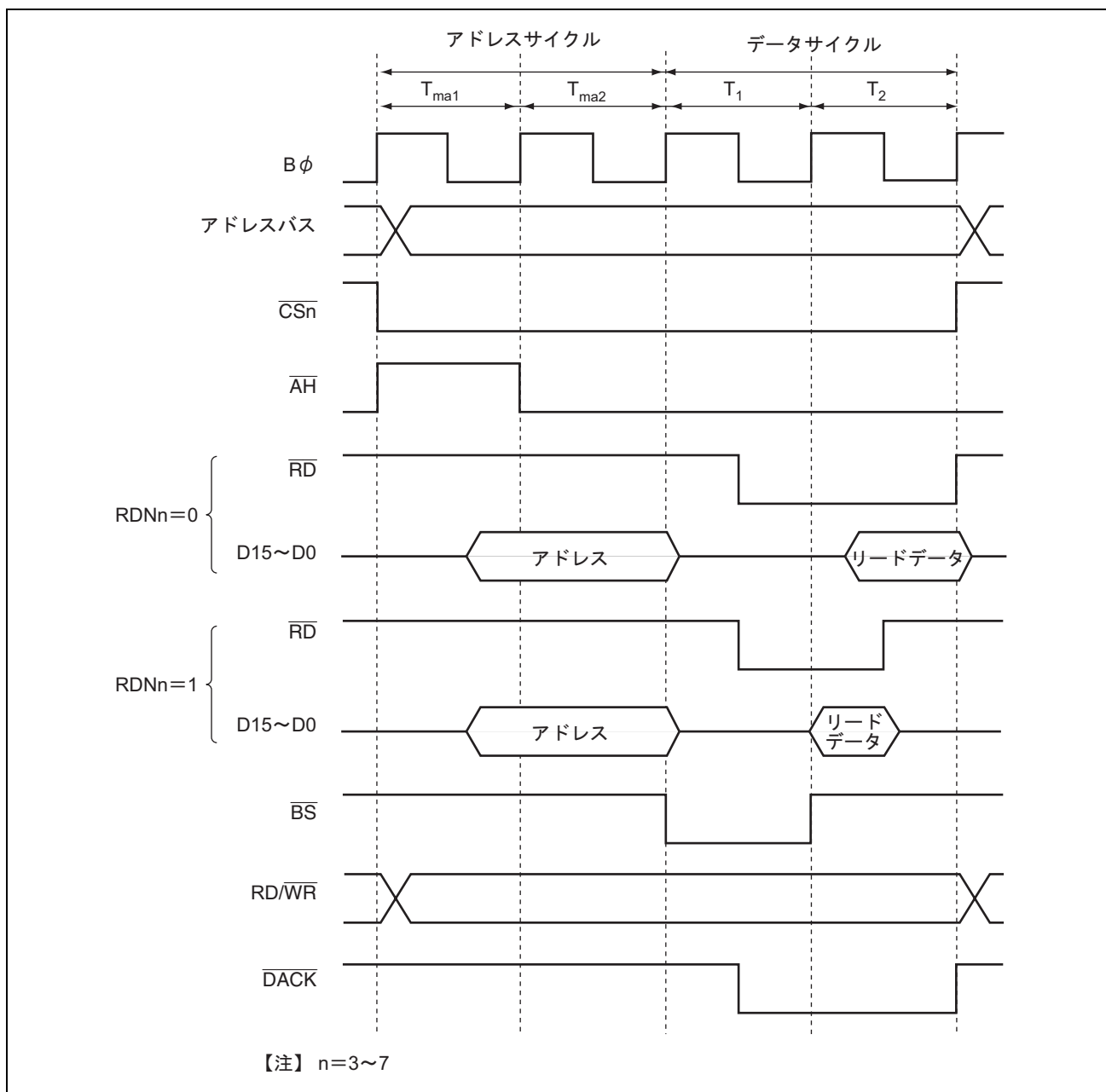
図 9.33 リードストローブタイミング例
