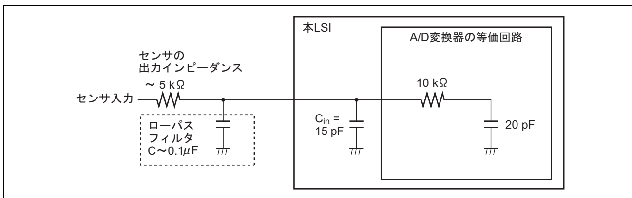
図 19.12 アナログ入力回路の例
