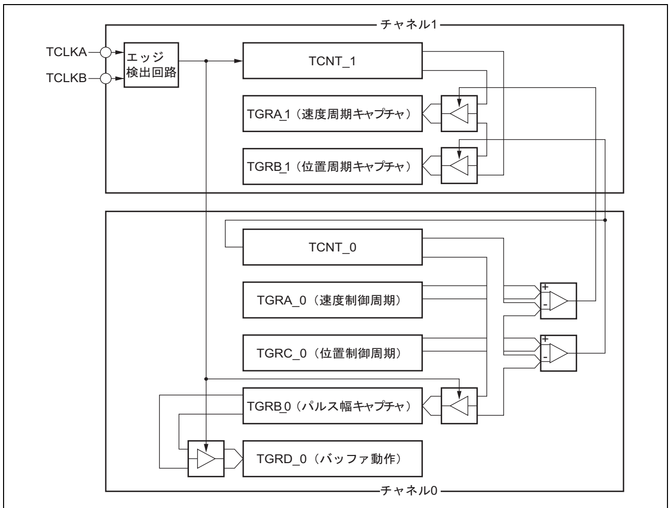
図 13.30 位相計数モードの応用例
