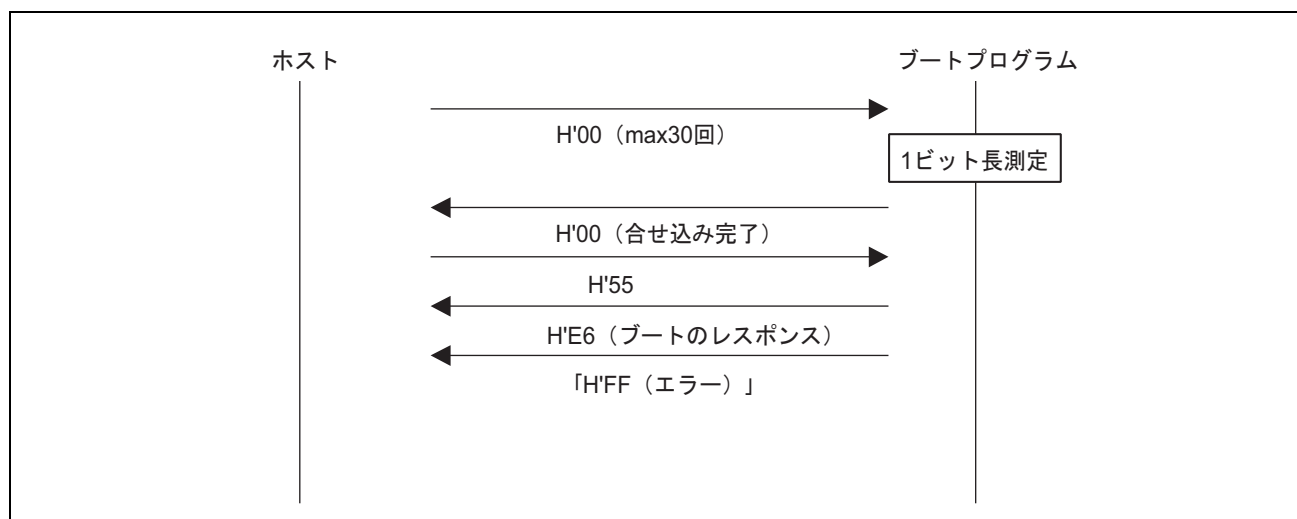
図 22.22 ビットレート合わせ込みのシーケンス
