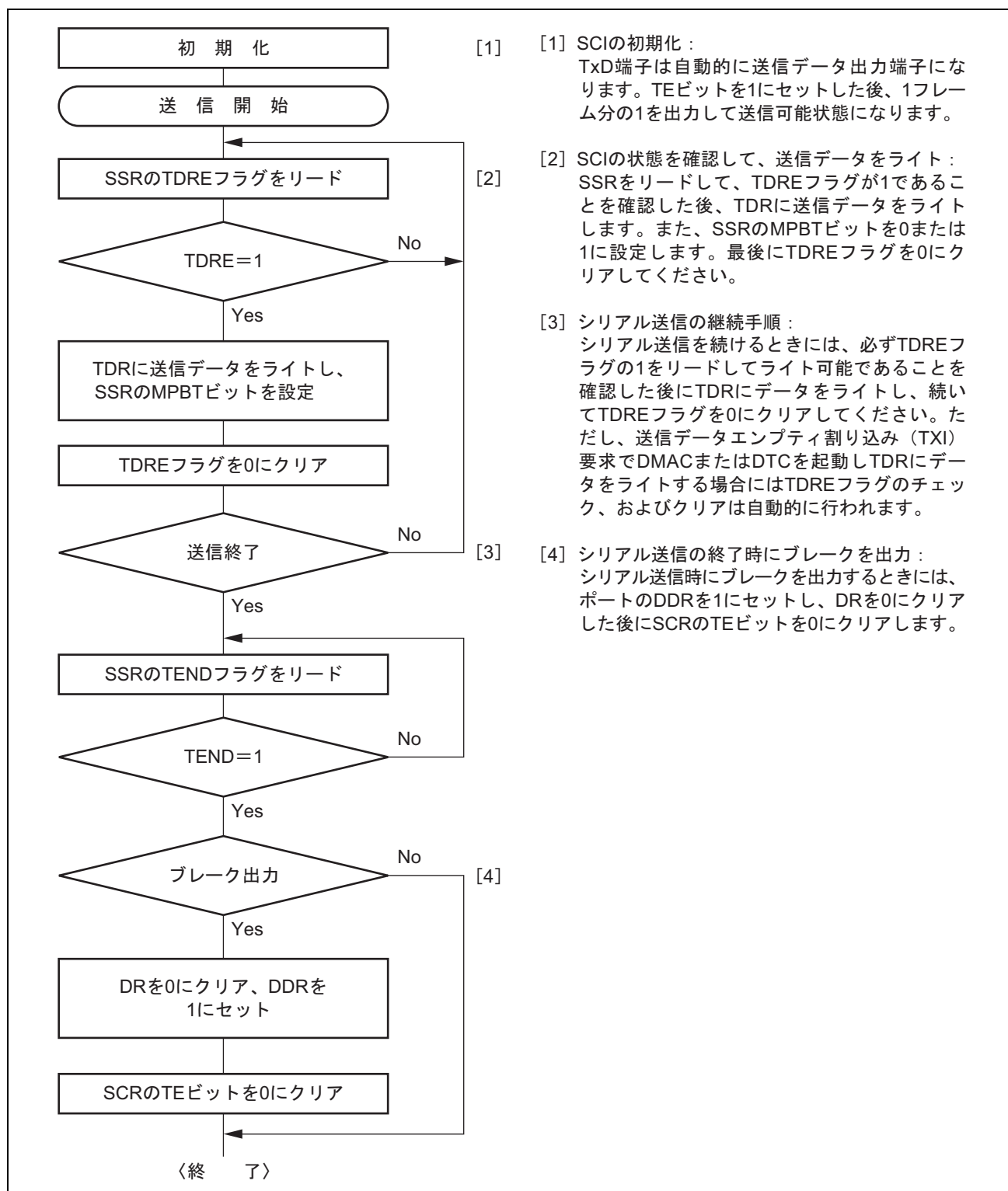
図 17.14 マルチプロセッサシリアル送信のフローチャートの例
