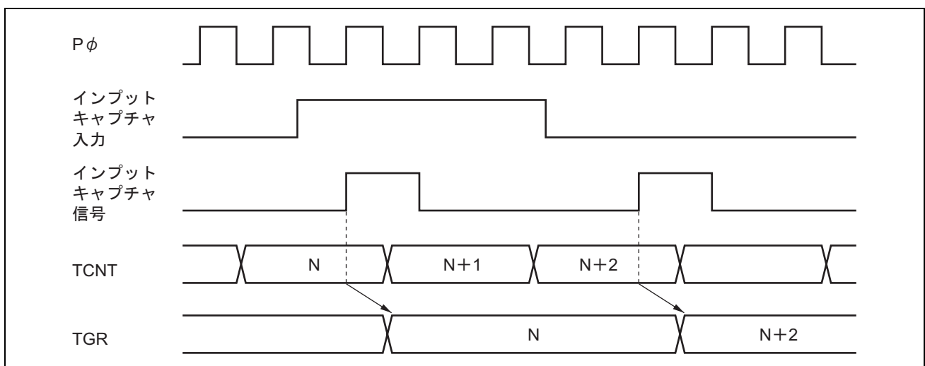
図 13.34 インพุットキャプチャ入力信号タイミング
