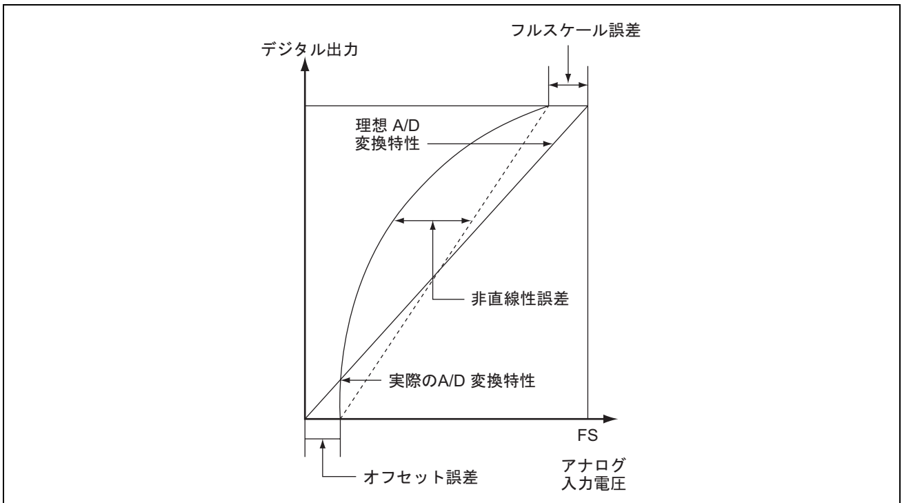
図 19.10 A/D 変換精度の定義
