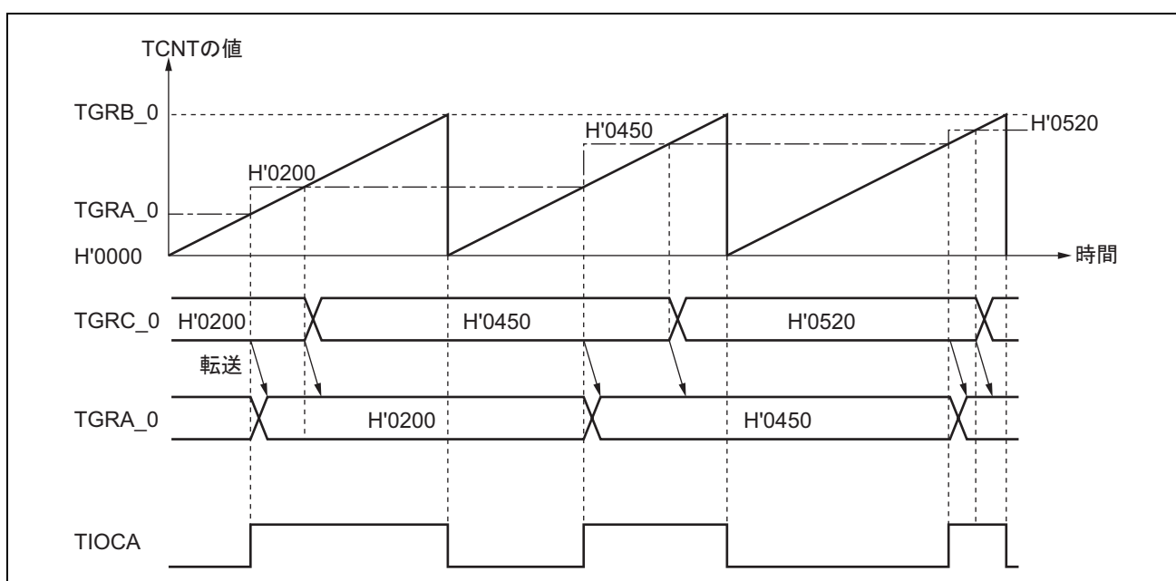
図 13.16 バッファ動作例 (1)
