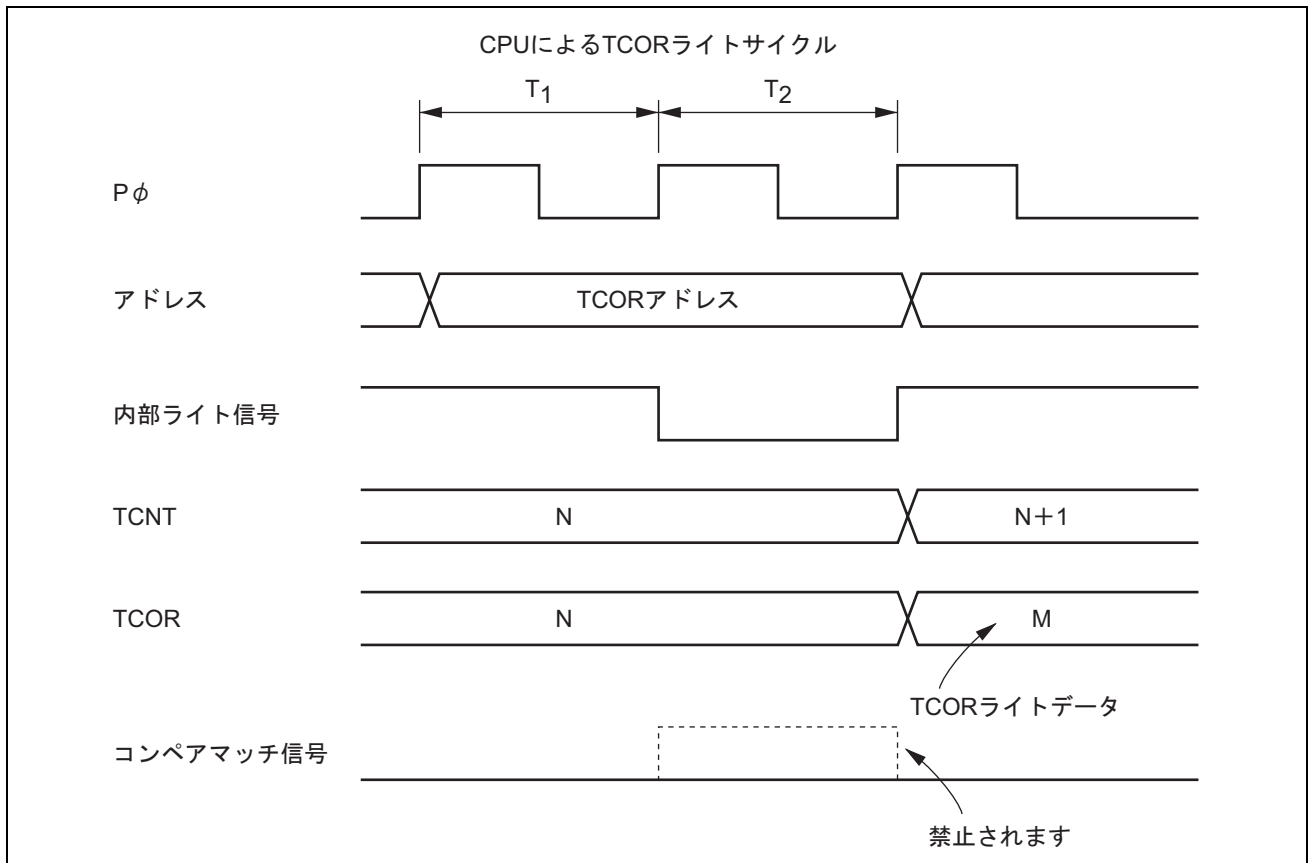
図 15.17 TCORのライトとコンペアマッチの競合
