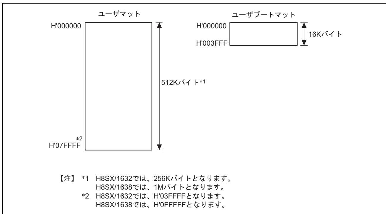
図 22.3 メモリマツト構成 (H8SX/1634)
