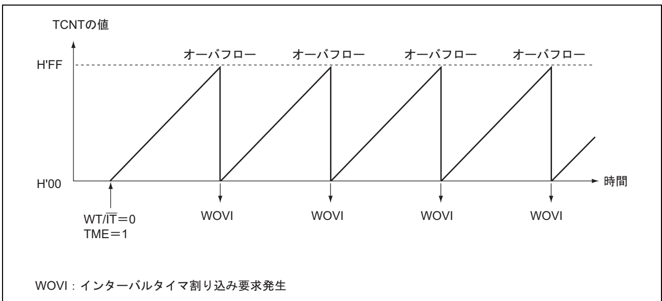
図 16.3 インターバルタイマモード時の動作
