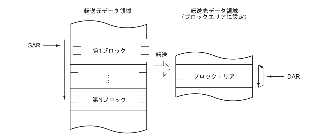
図 11.9 ブロック転送モードのメモリマップ（転送先をブロックエリアに指定した場合）
