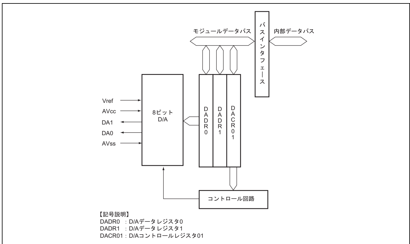
図 20.1 D/A 変換器のブロック図
