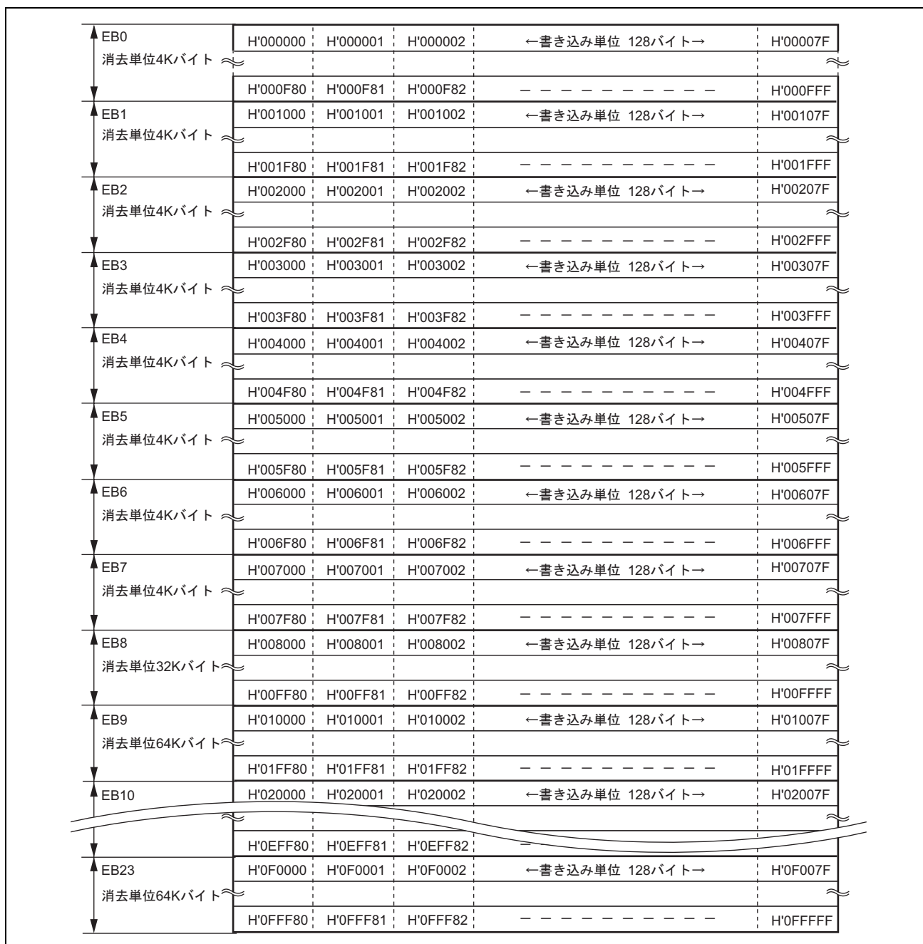
図 22.4 (3) H8SX/1638 のユーザマットのブロック構成
