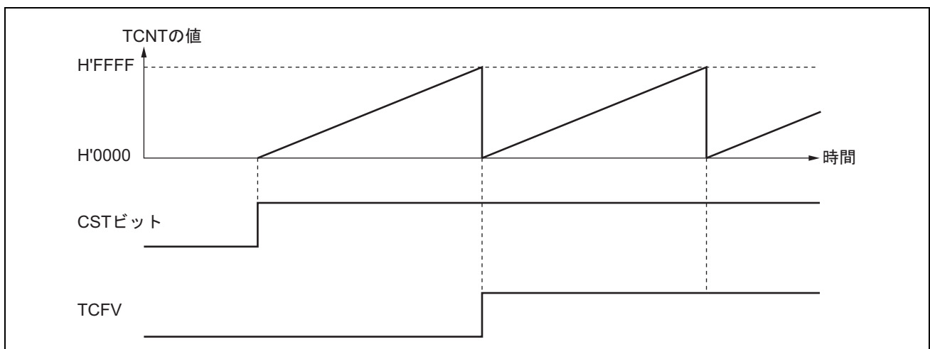
図 13.4 フリーランニングカウンタの動作
