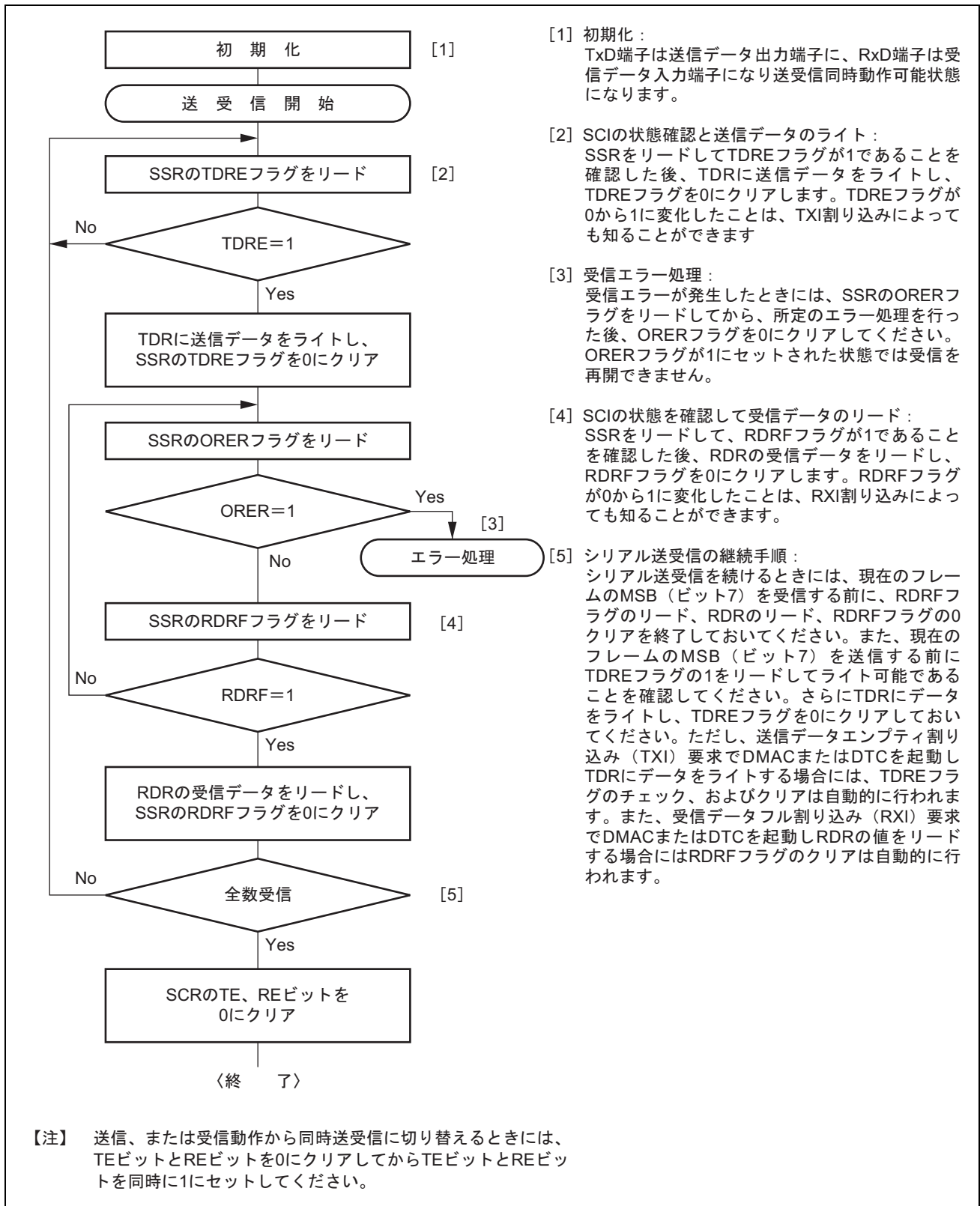
図 17.23 シリアル送受信同時動作のフローチャートの例
