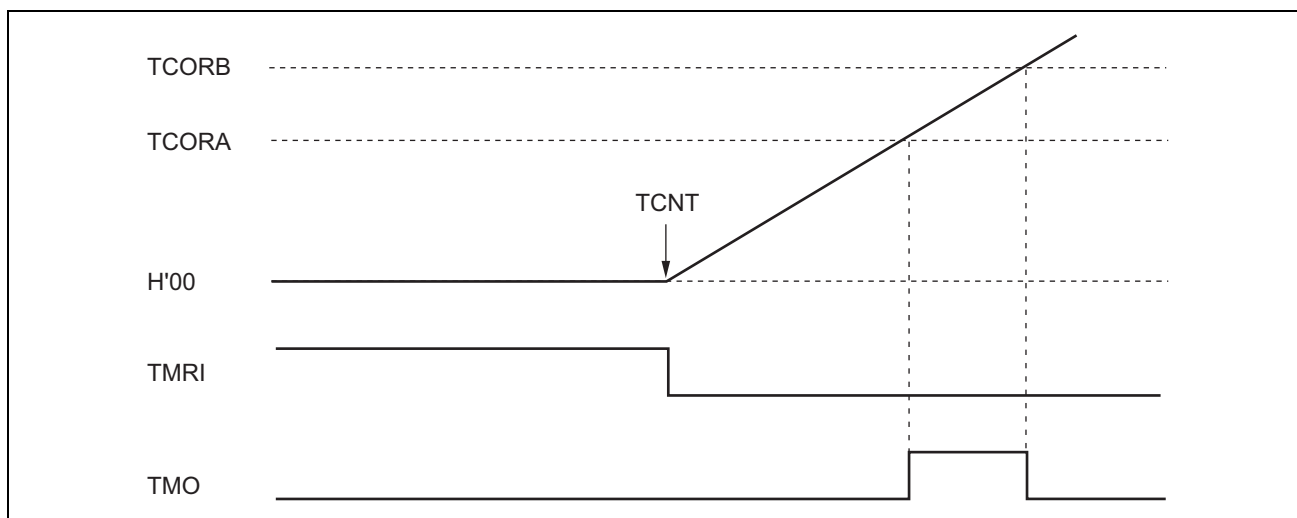
図 15.6 リセット入力例
