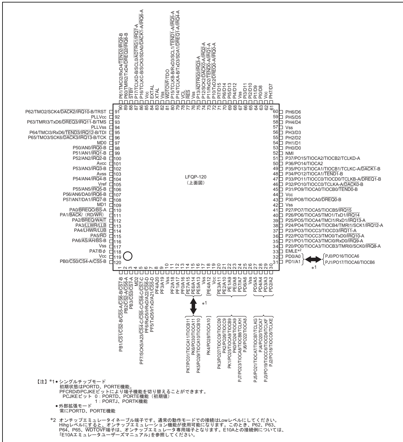
図 1.3 ピン配置図
