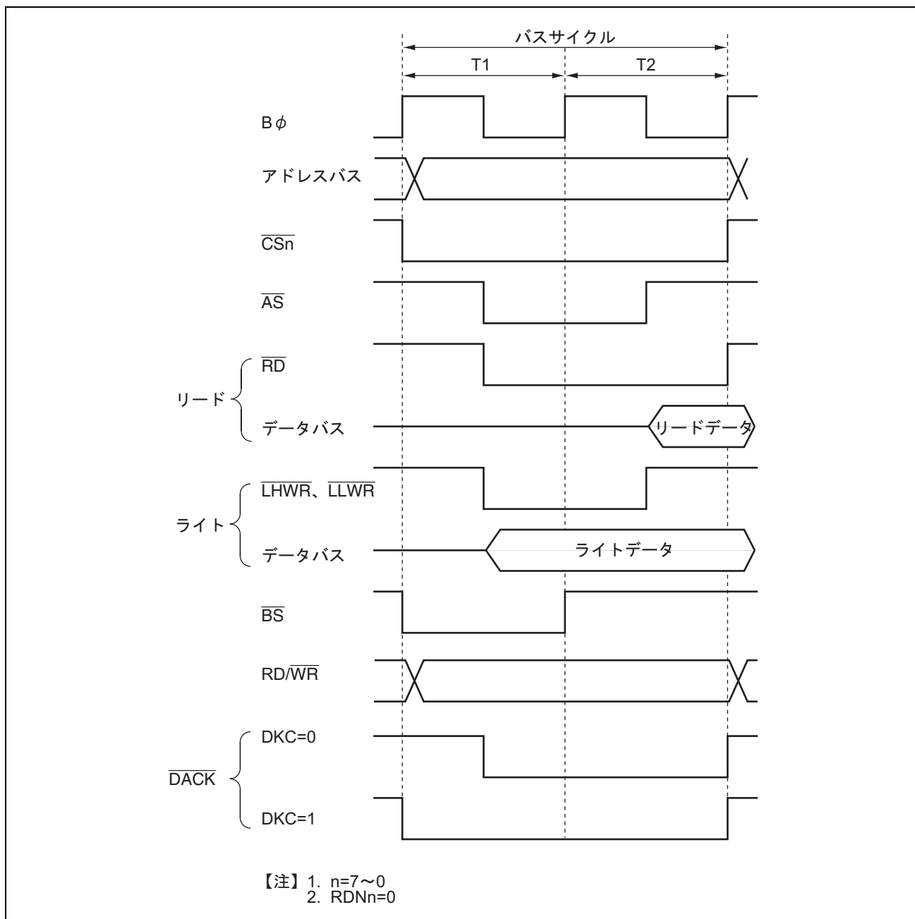
図 9.23 \overline{\text{DACK}} 信号の出力タイミング
