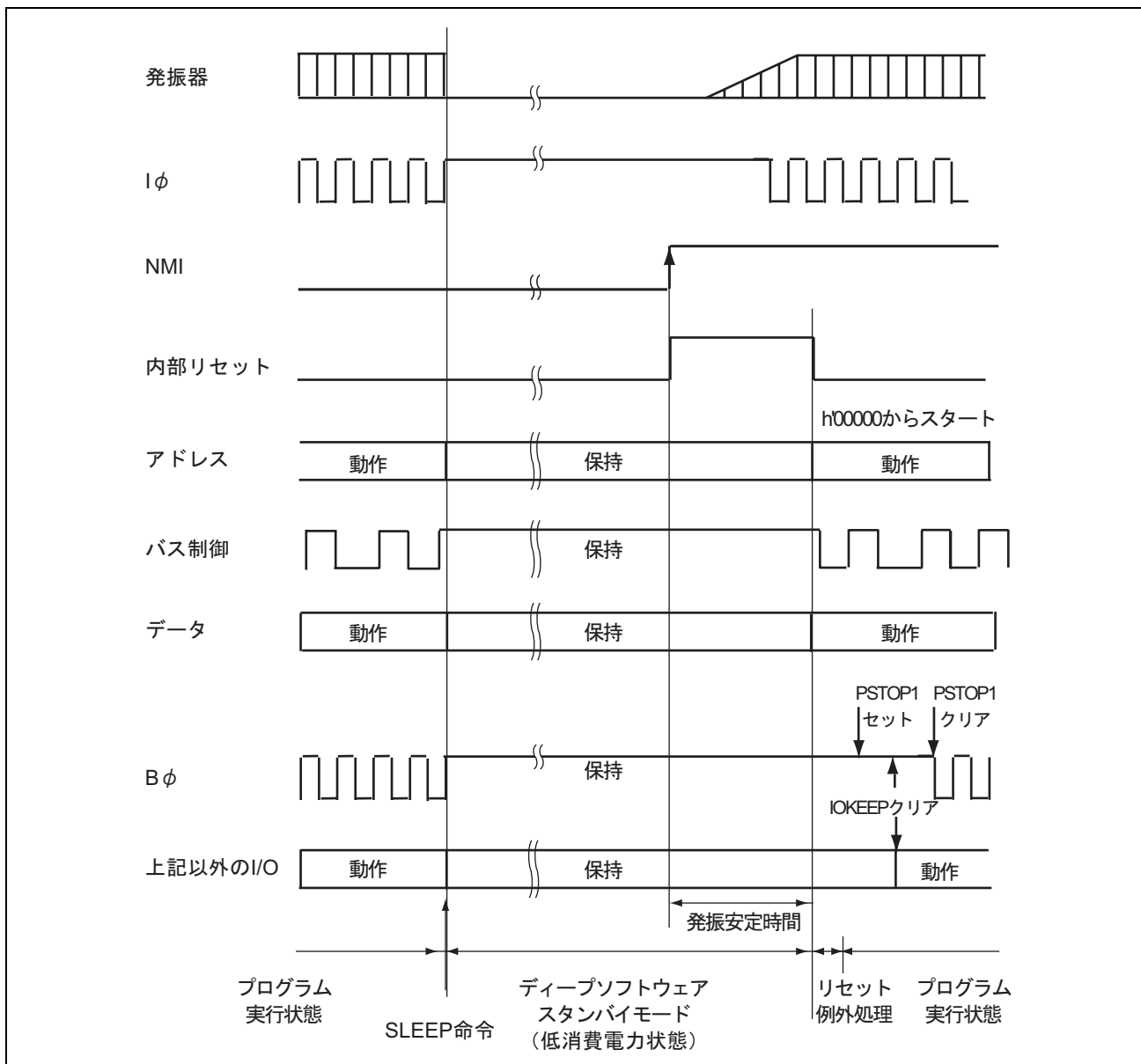
図 25.5 外部拡張モード時のディープソフトウェアスタンバイモードの動作例 (IOKEEP=OPE=1 のとき)
