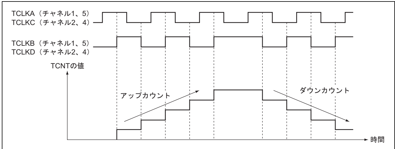
図 13.29 位相計数モード4の動作例
