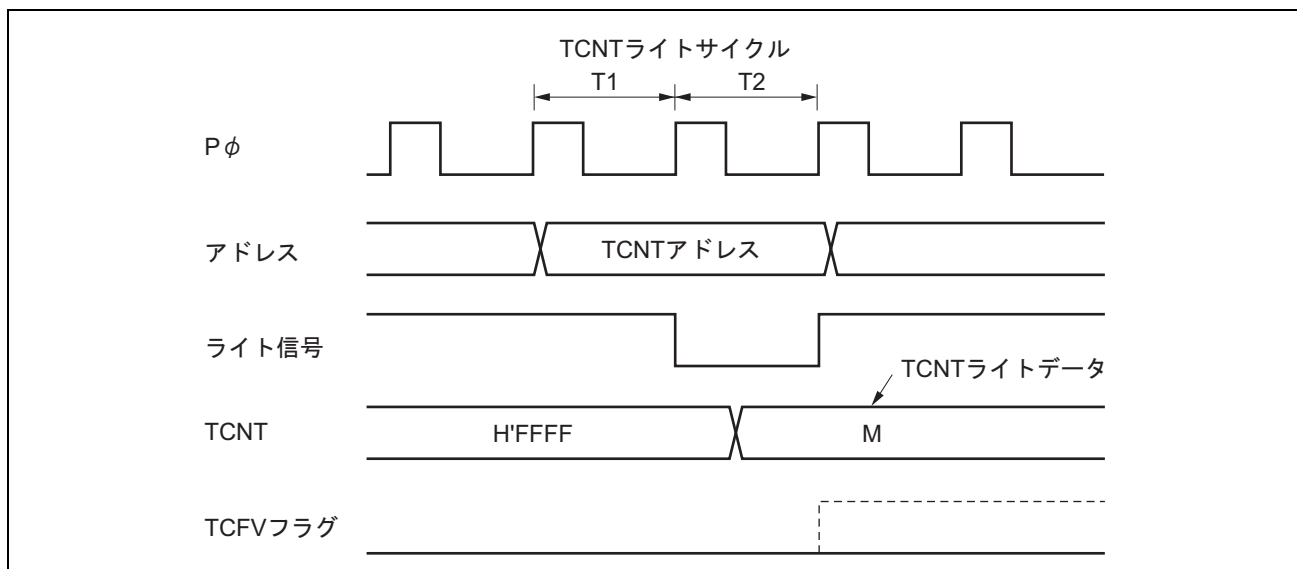
図 13.55 TCNT のライトとオーバフローの競合
