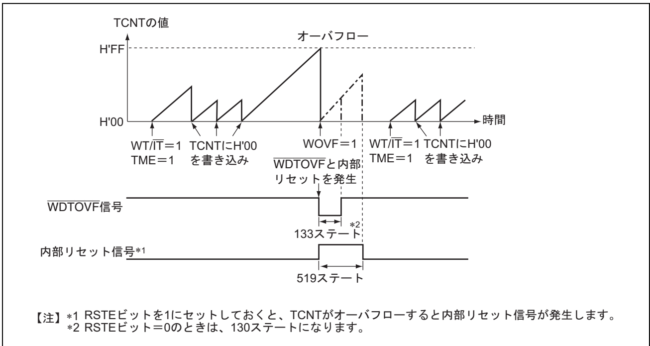
図 16.2 ウォッチドッグタイマモード時の動作
