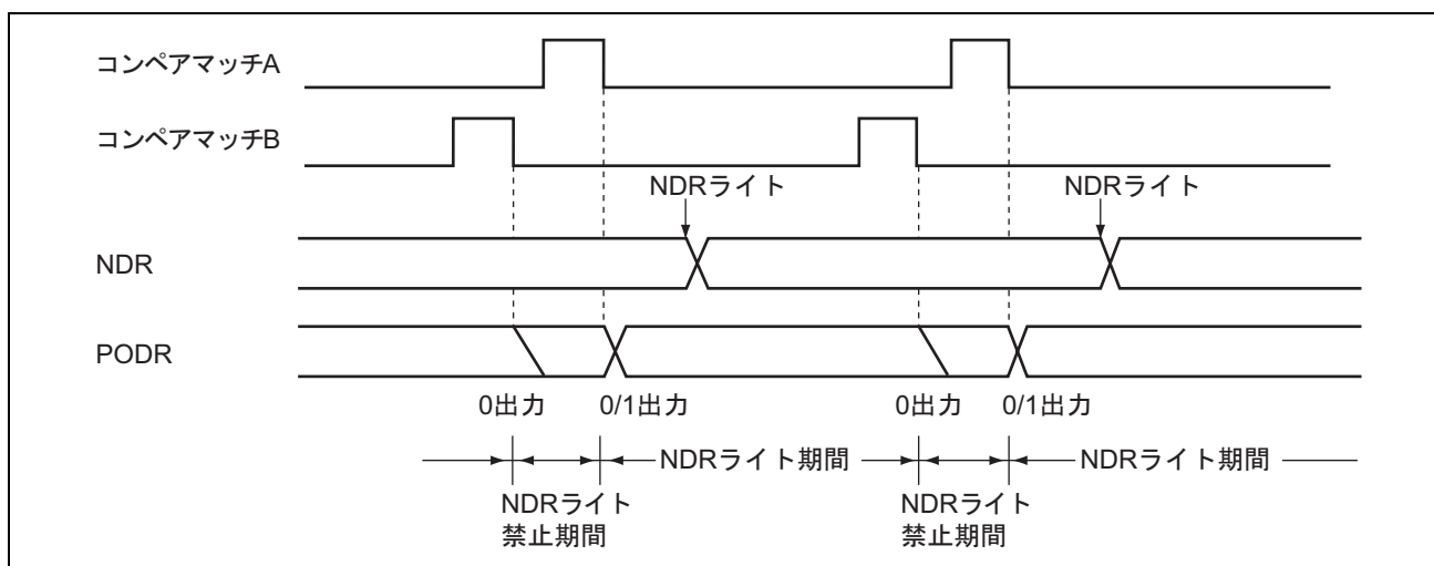
図 14.9 ノンオーバーラップ動作と NDR ライトタイミング
