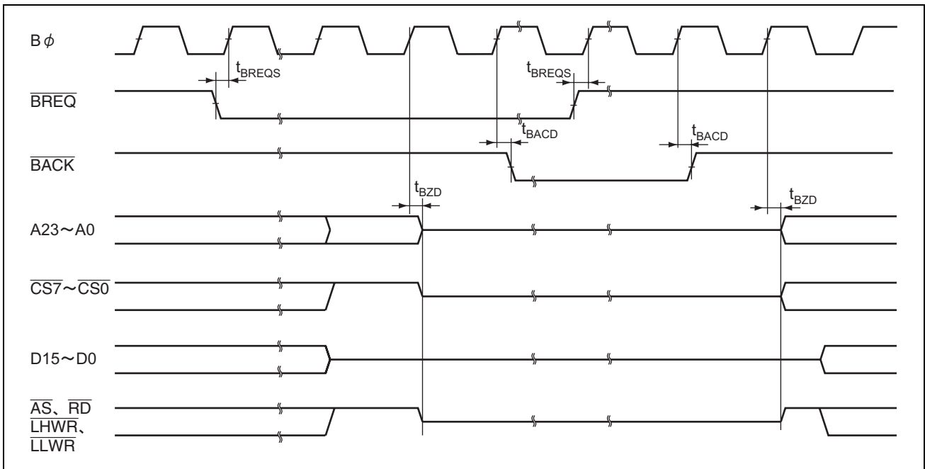
図 27.19 外部バス権開放タイミング
