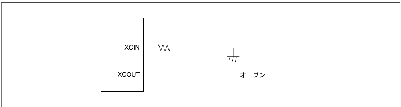
図 9.10 サブクロック発振器を使用しない場合の端子処理
