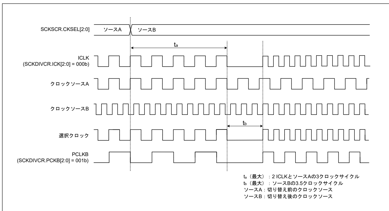
図 9.19 クロックソース切り替えのタイミング
