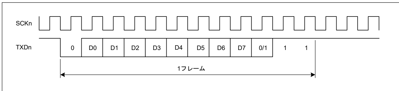
図 26.4 調歩同期式モードにおける出力クロックと送信データの位相関係 (SMR.CHR = 0、PE = 1、MP = 0、および STOP = 1 の場合)
