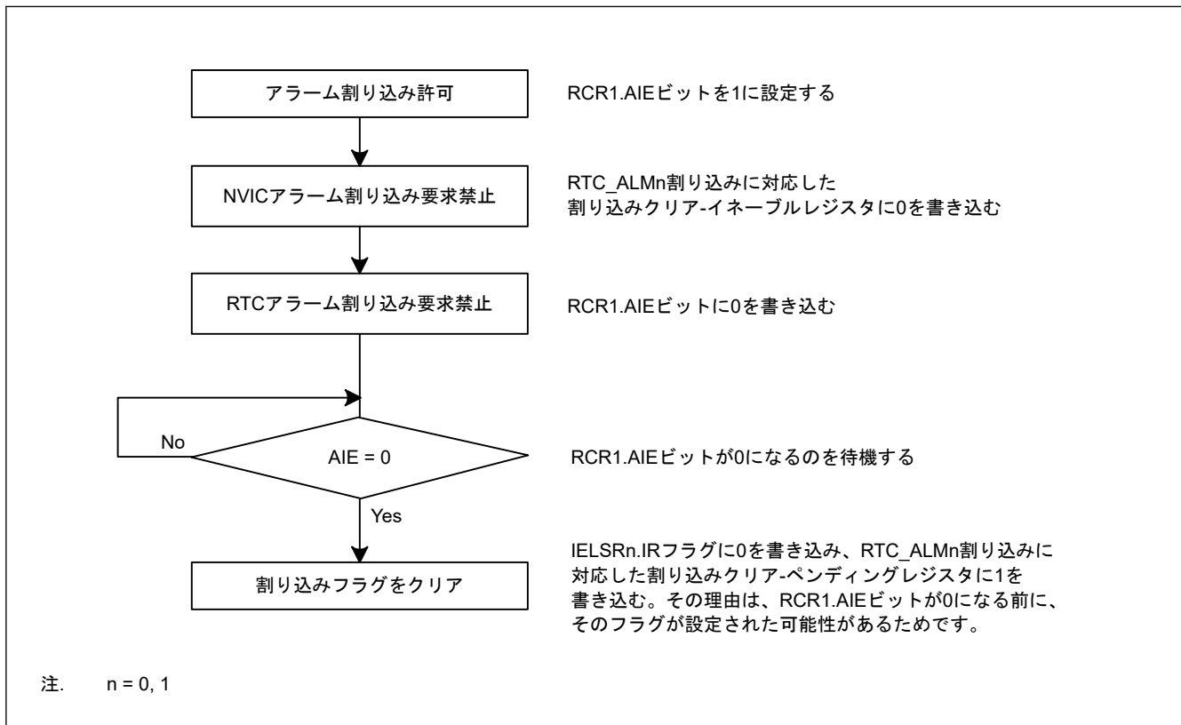
図 23.9 アラーム割り込み要求の禁止手順
