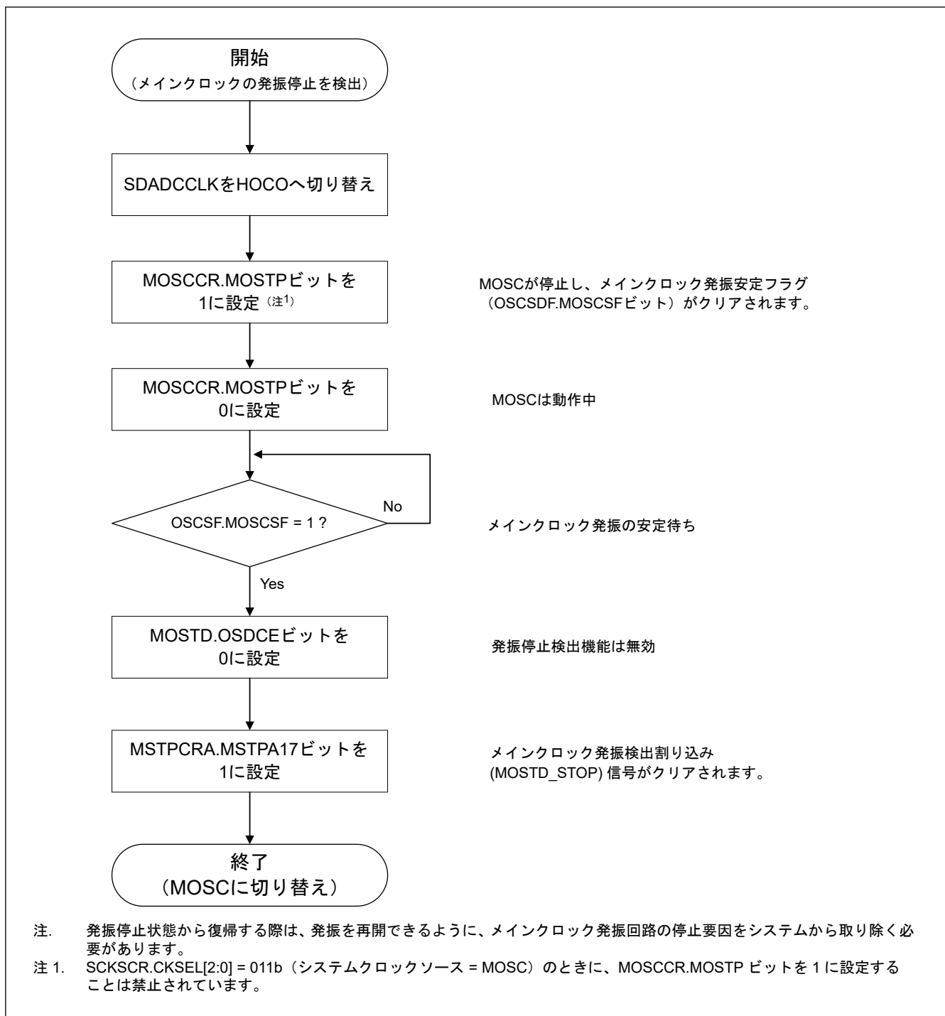
図 9.17 メインクロック発振器停止検出による SDADCCLK クロックソース切り替え後の復帰手順
