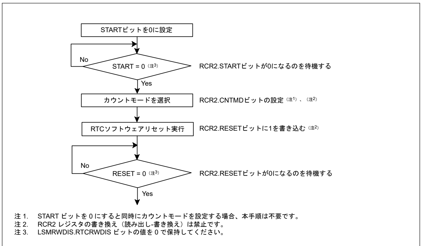
図 23.3 クロックおよびカウントモードの設定手順
