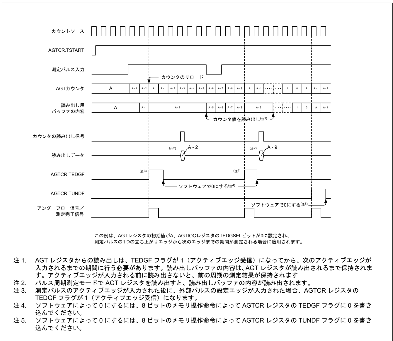
図 21.11 パルス周期測定モードでの動作例
