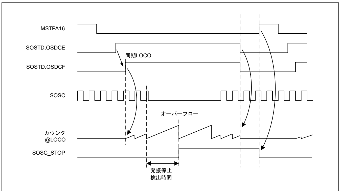
図 9.12 サブクロック発振停止検出器による発振停止検出のタイミング
