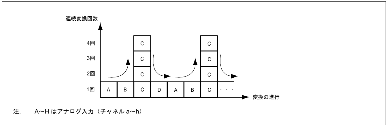
図 30.2 ADADC.ADC[2:0] = 011b および ADADS0 によるアナログ入力 C を 1 に選択時のスキャン変換シーケンス
