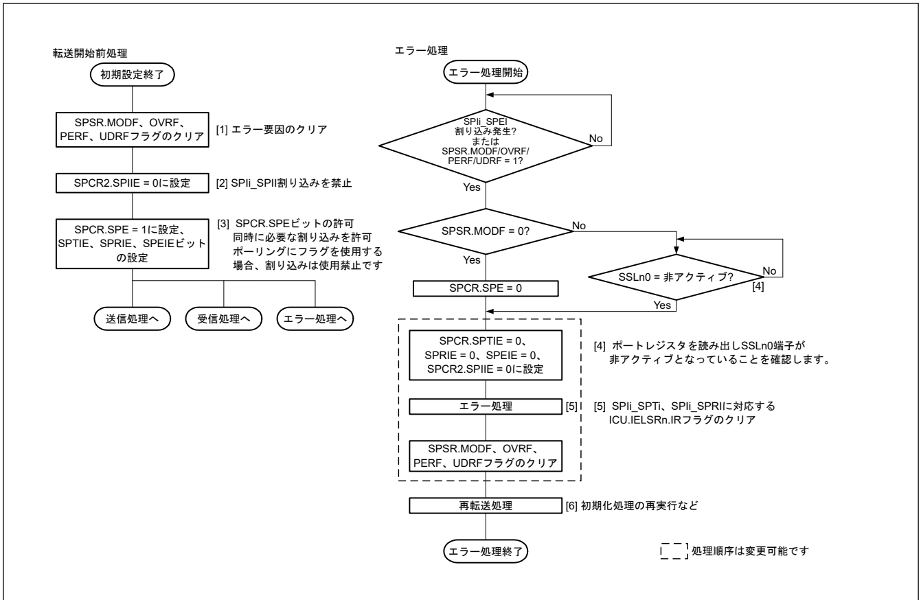
図 28.35 マスタモードでのエラー処理手順
