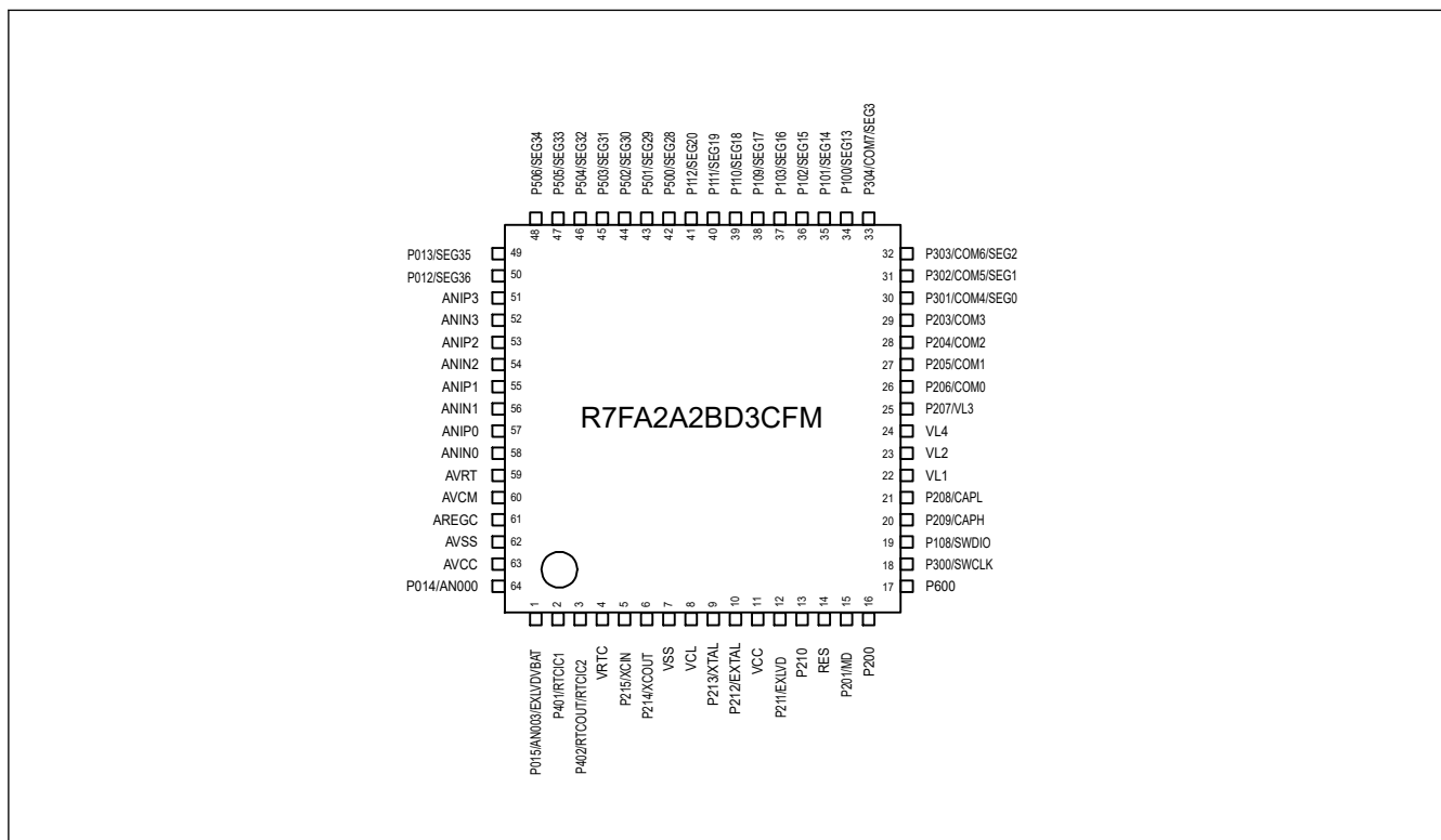
図 1.6 64 ピン LQFP のピン配置図 (上面図)
