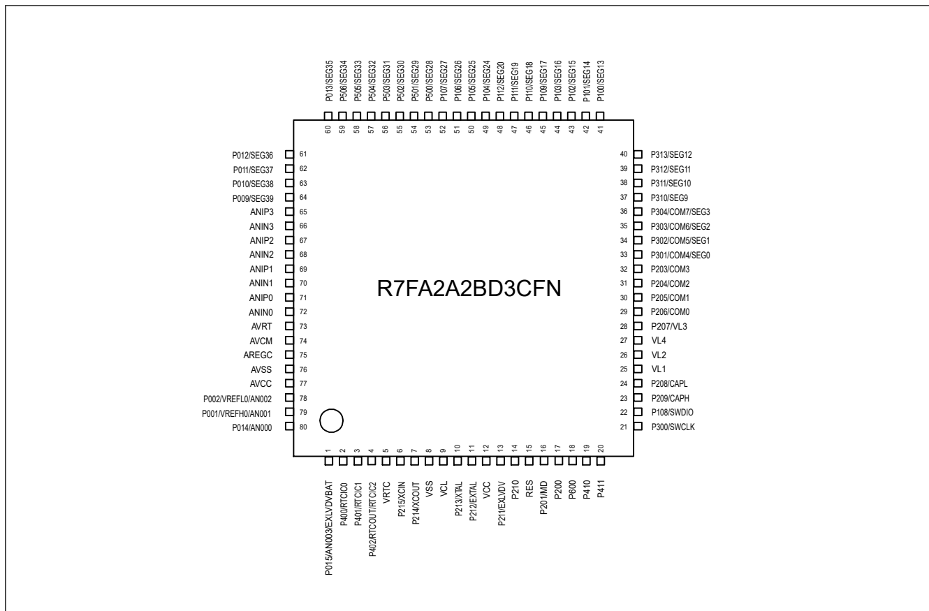
図 1.5 80 ピン LQFP のピン配置図 (上面図)
