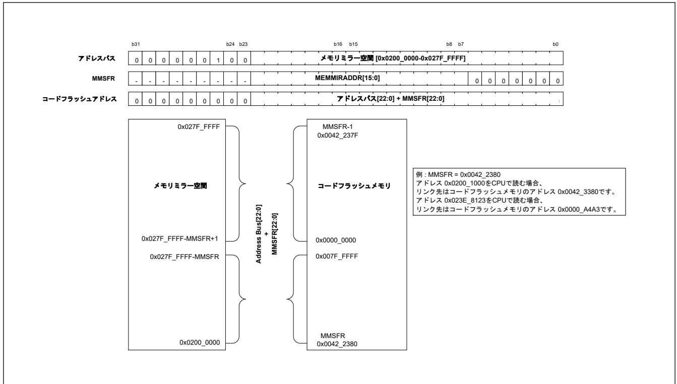
図 5.1 MMF の概要
