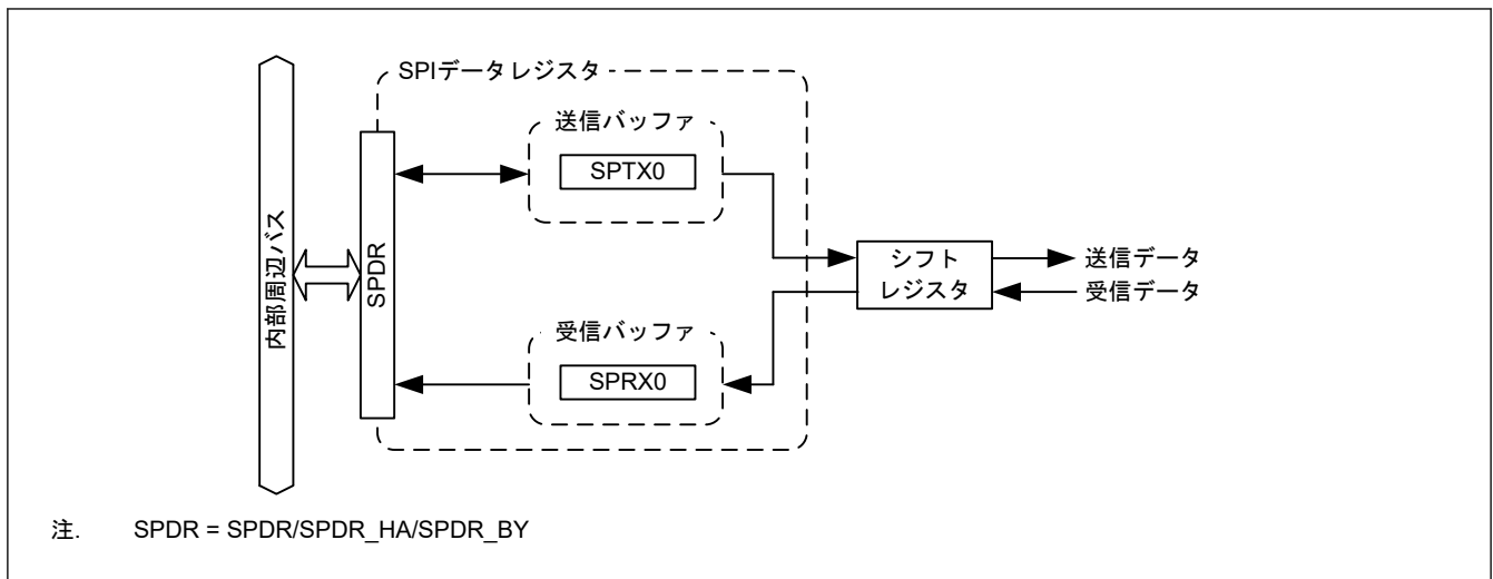
図 28.2 SPDR/SPDR_HA/SPDR_BY の構成
