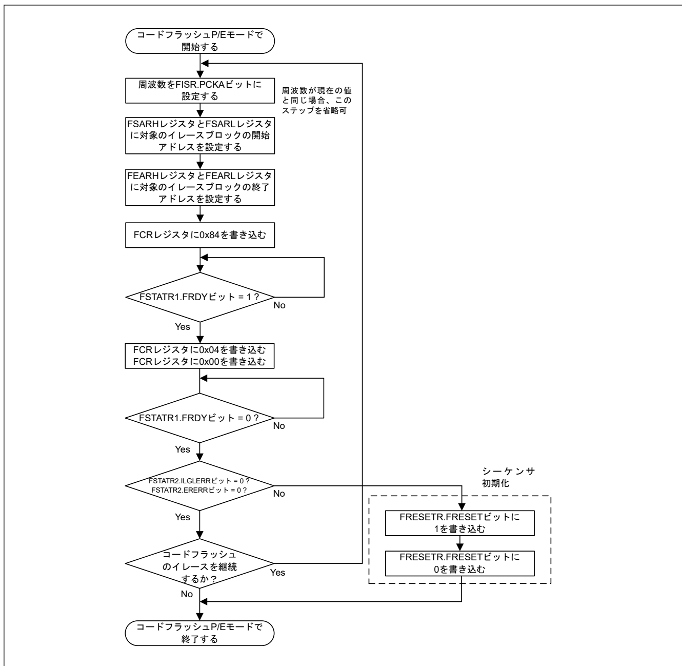
図 35.32 コードフラッシュブロックイレース手順のフローチャート
