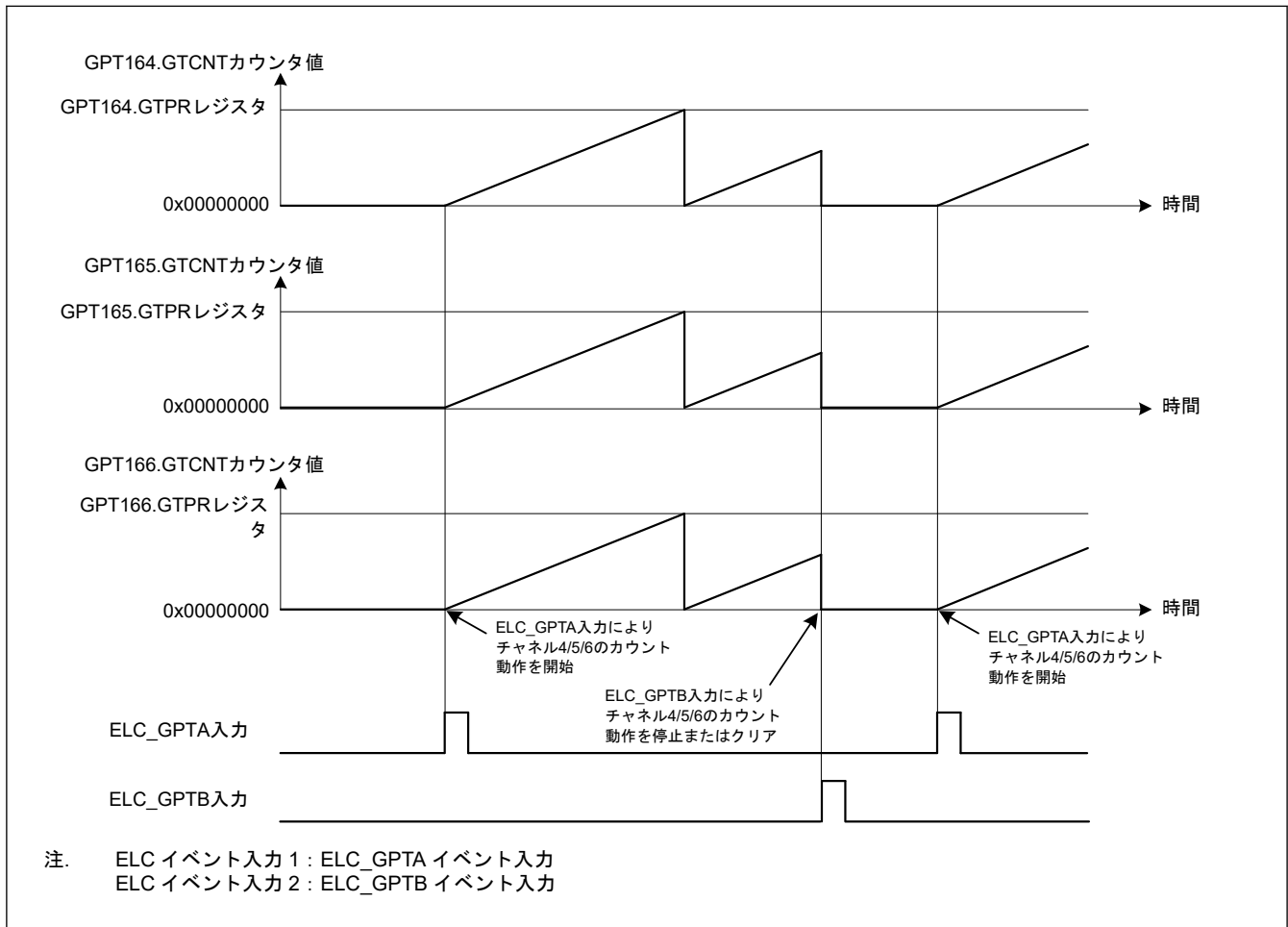
図 20.38 ハードウェア要因による同時スタート/ストップ/クリア動作例 (カウント周期 (GTPR レジスタ値) が同一のとき)
