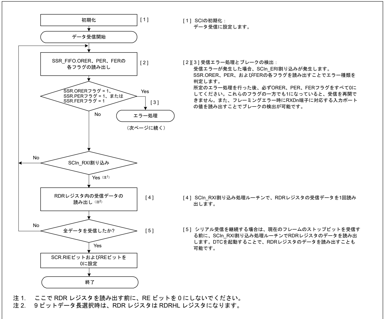
図 26.15 調歩同期式モードにおけるシリアル受信のフローチャート例（非 FIFO 選択、アドレス一致検出無効時）(1)
