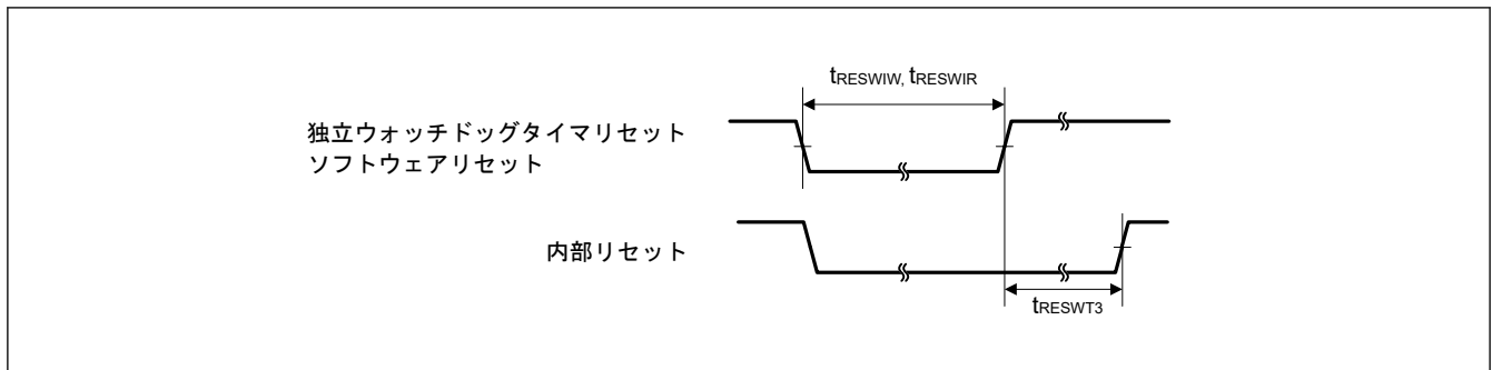
図 41.10 リセット入カタイミング (2)
