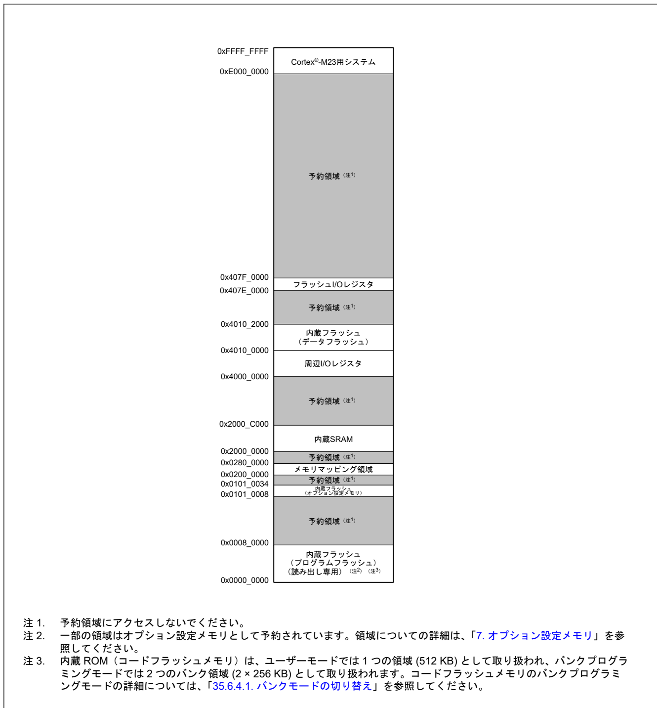
図 4.1 メモリマップ
