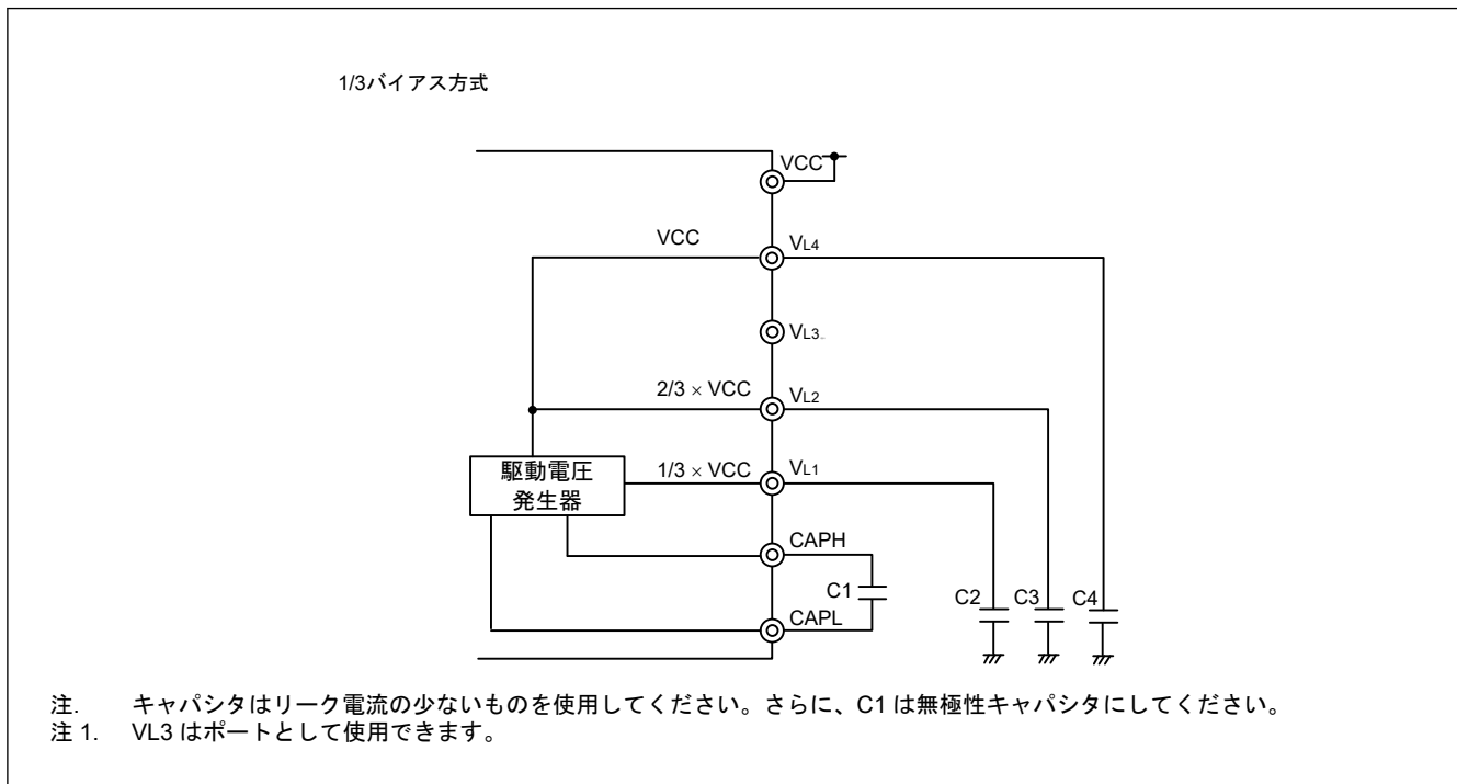
図 36.14 容量分割方式の VCC 基準モードを使用する LCD 駆動電源接続の例
