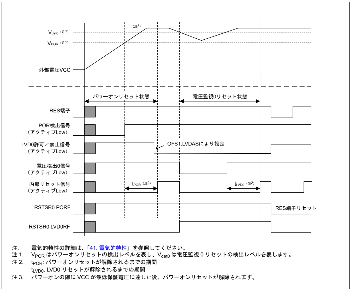
図 8.7 電圧監視 0 リセットの動作例
