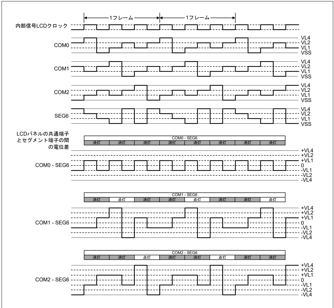
図 36.31 1/3 バイアス方式を使用時の SEG6 と各共通信号の間の 3 タイムスライス LCD 駆動波形の例
