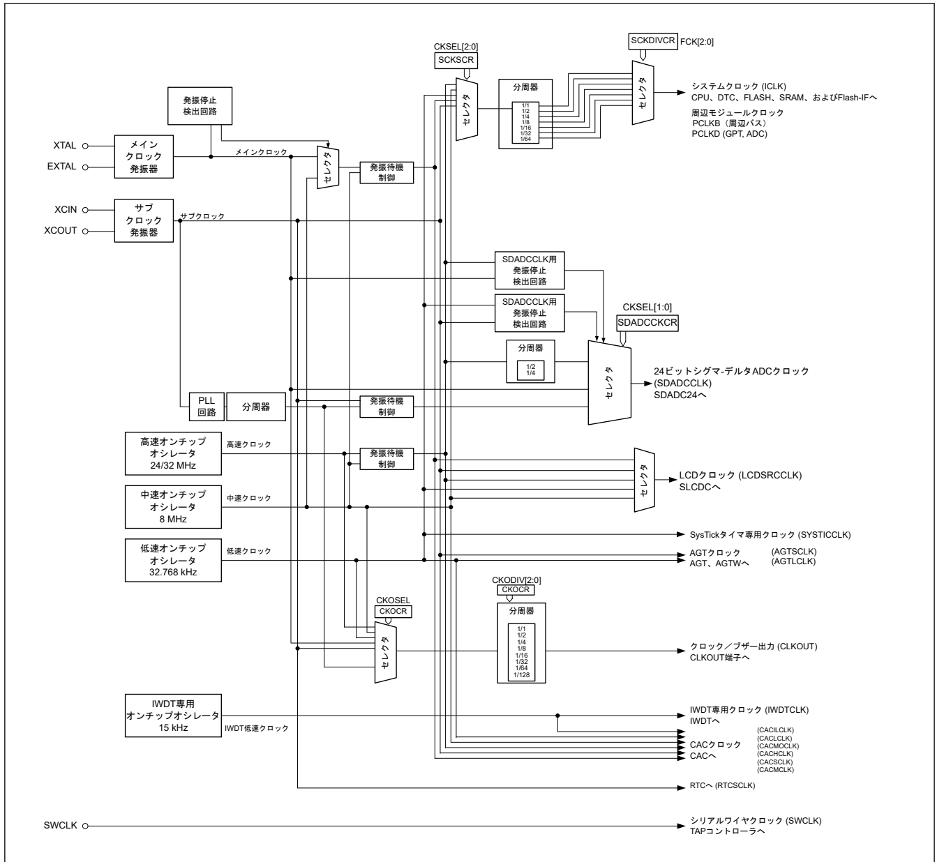
図 9.2 クロック発生回路のブロック図 (内部クロック供給先アーキテクチャ B)
