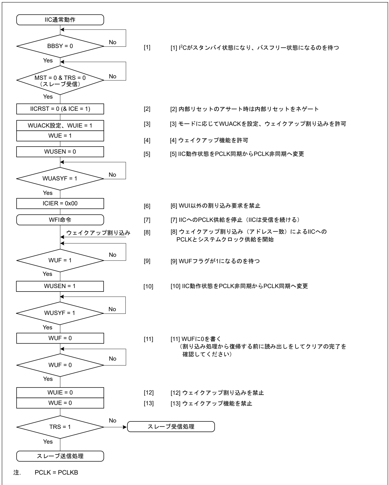
図 27.33 ノーマルウェイクアップモード2の動作例 (スレーブアドレス一致時のウェイクアップ割り込みによるウェイクアップの場合)
