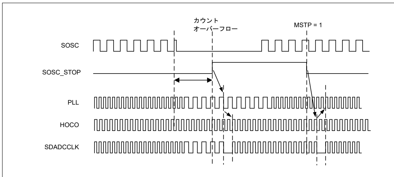
図 9.13 SDADCCLK (SOSC 停止検出) のクロックソース切り替えのタイミング
