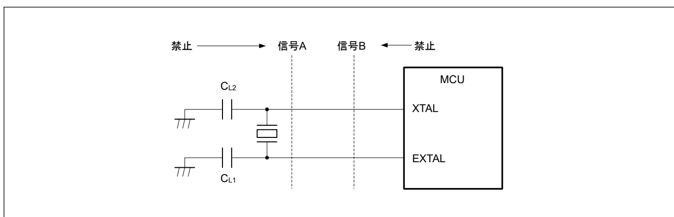
図 9.20 発振回路部のボード設計に関する信号のルーティング
