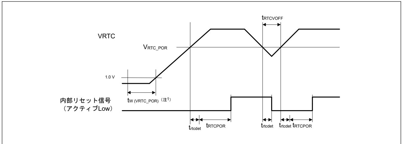
図 41.47 VRTC の電圧検出リセットタイミングとパワーオンリセットタイミング
