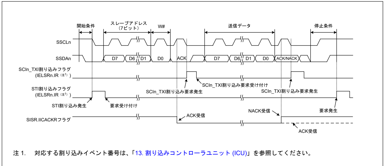
図 26.63 簡易 IIC モードにおけるマスタ送信の動作例 1 (7 ビットスレーブアドレス、送信割り込み、受信割り込み使用時)
