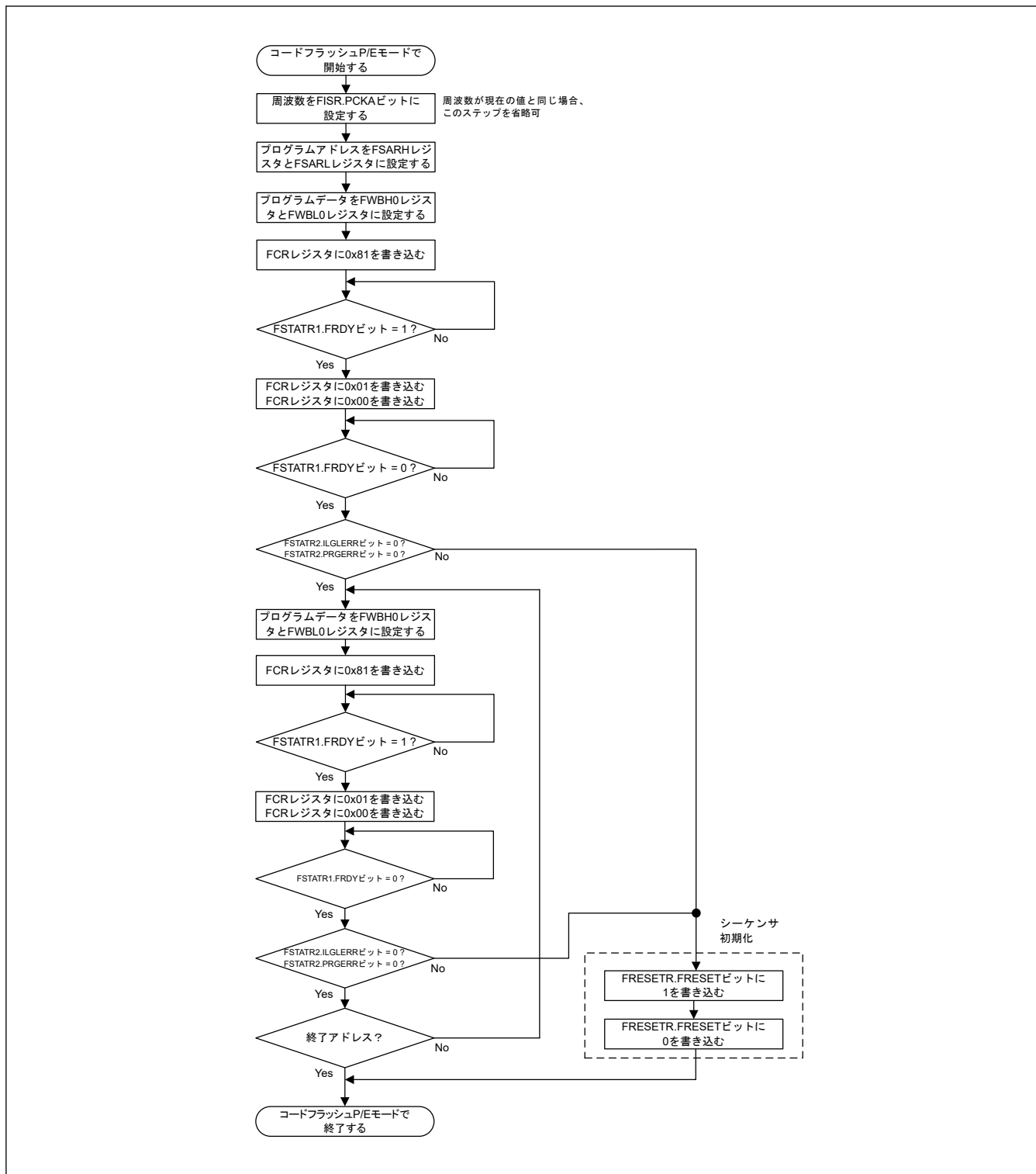
図 35.30 コードフラッシュの連続プログラム時のフローチャート
