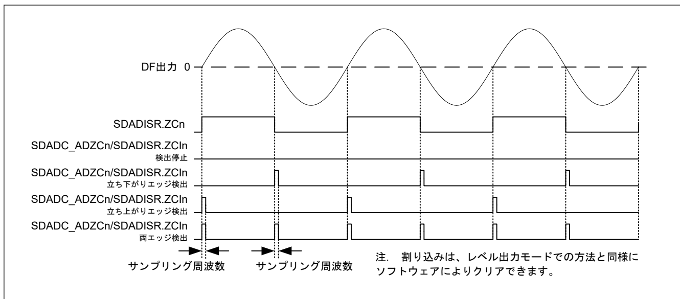
図 31.10 SDADC_ADZCn 割り込み発生タイミング (パルス出力 : SDADICR.ZCMDn = 0)
