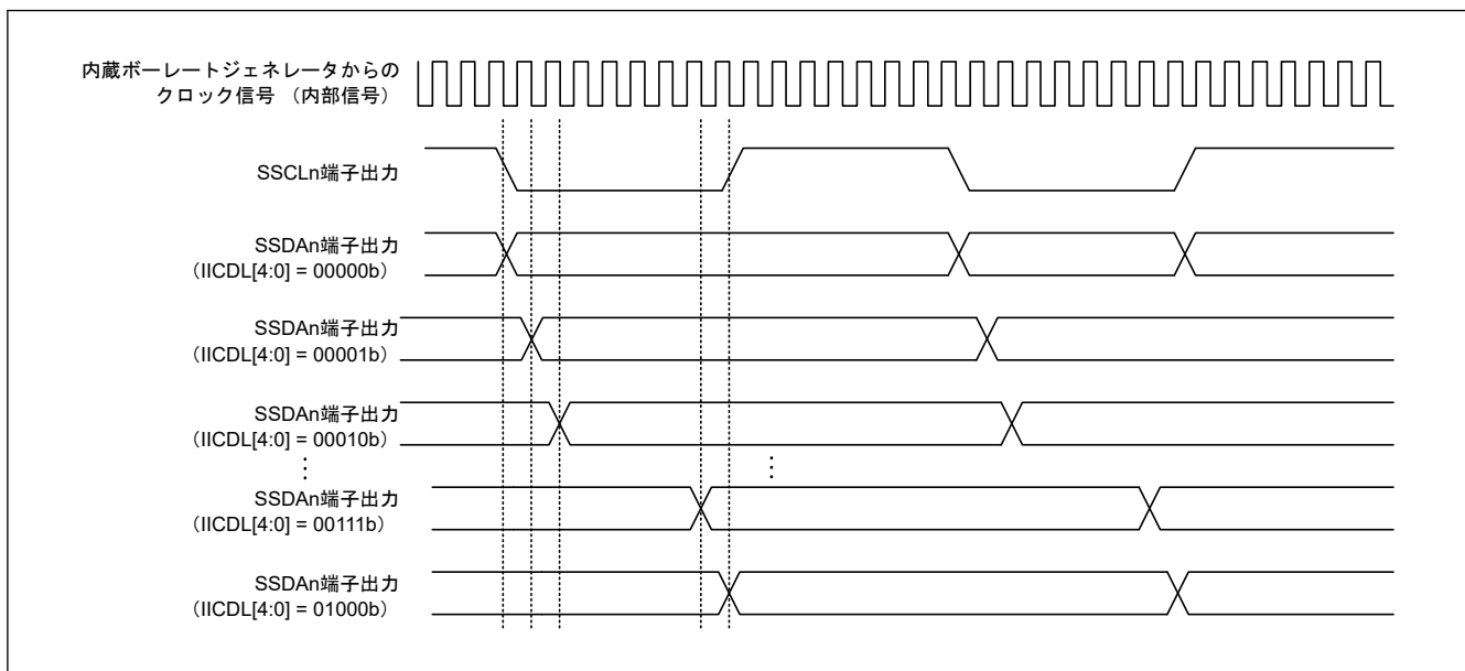
図 26.62 SDAn 出力遅延のタイミング
