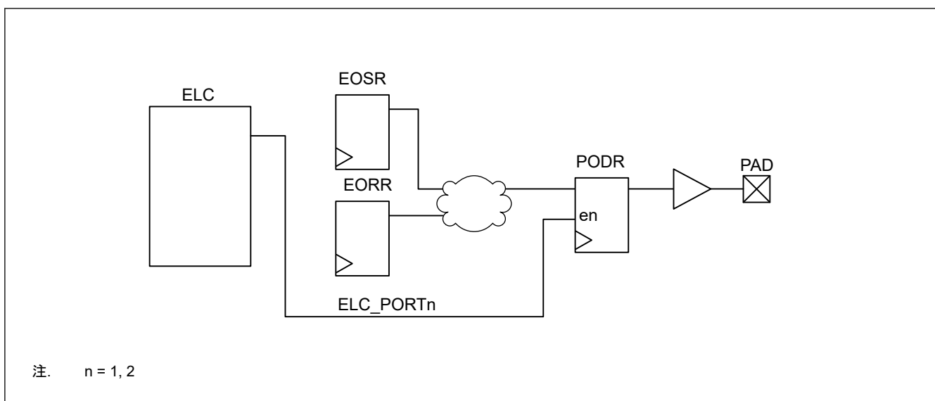
図 17.3 イベントポート出力データ
