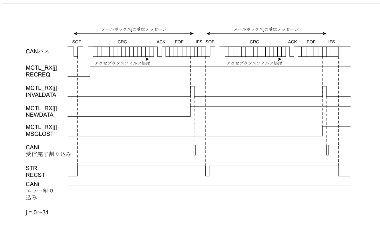
図 27.18 オーバーライトモードでのデータフレーム受信の動作例
