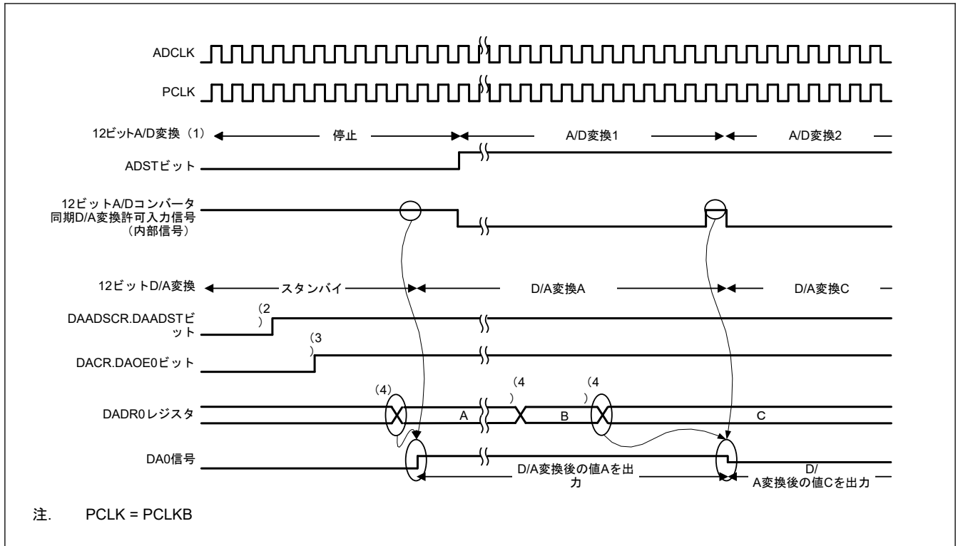
図 31.3 DAC12 を次に同期して変換する例：ADC12
