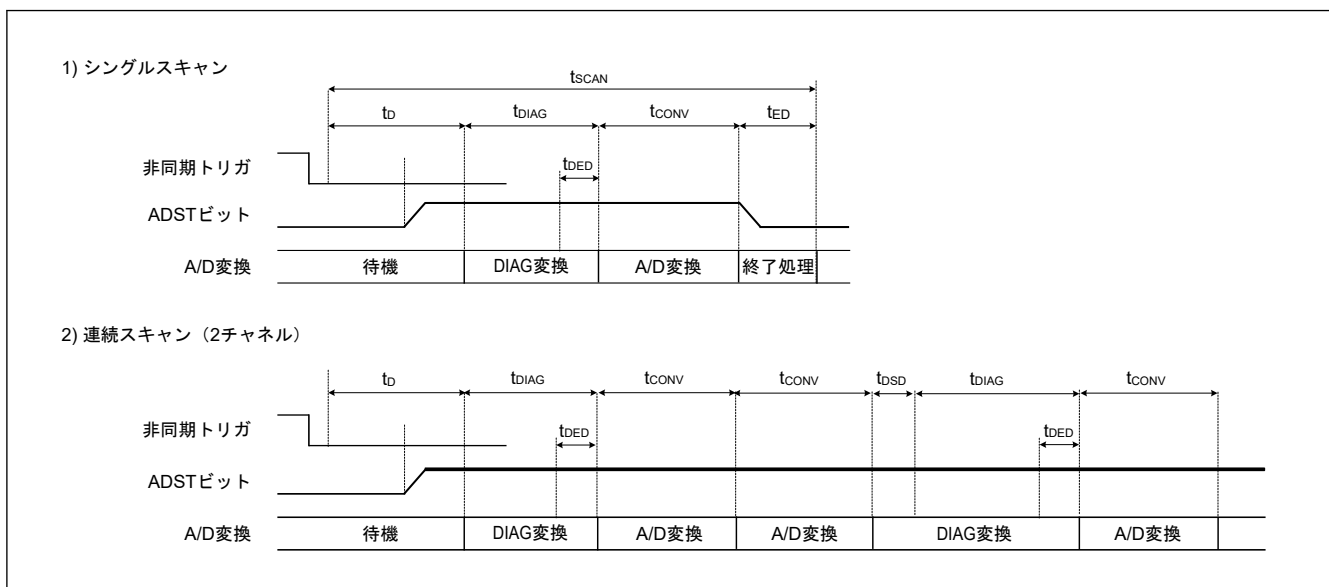
図 30.26 スキャン変換のタイミング (非同期トリガ入力 (ADTRG0) 起動の場合)
