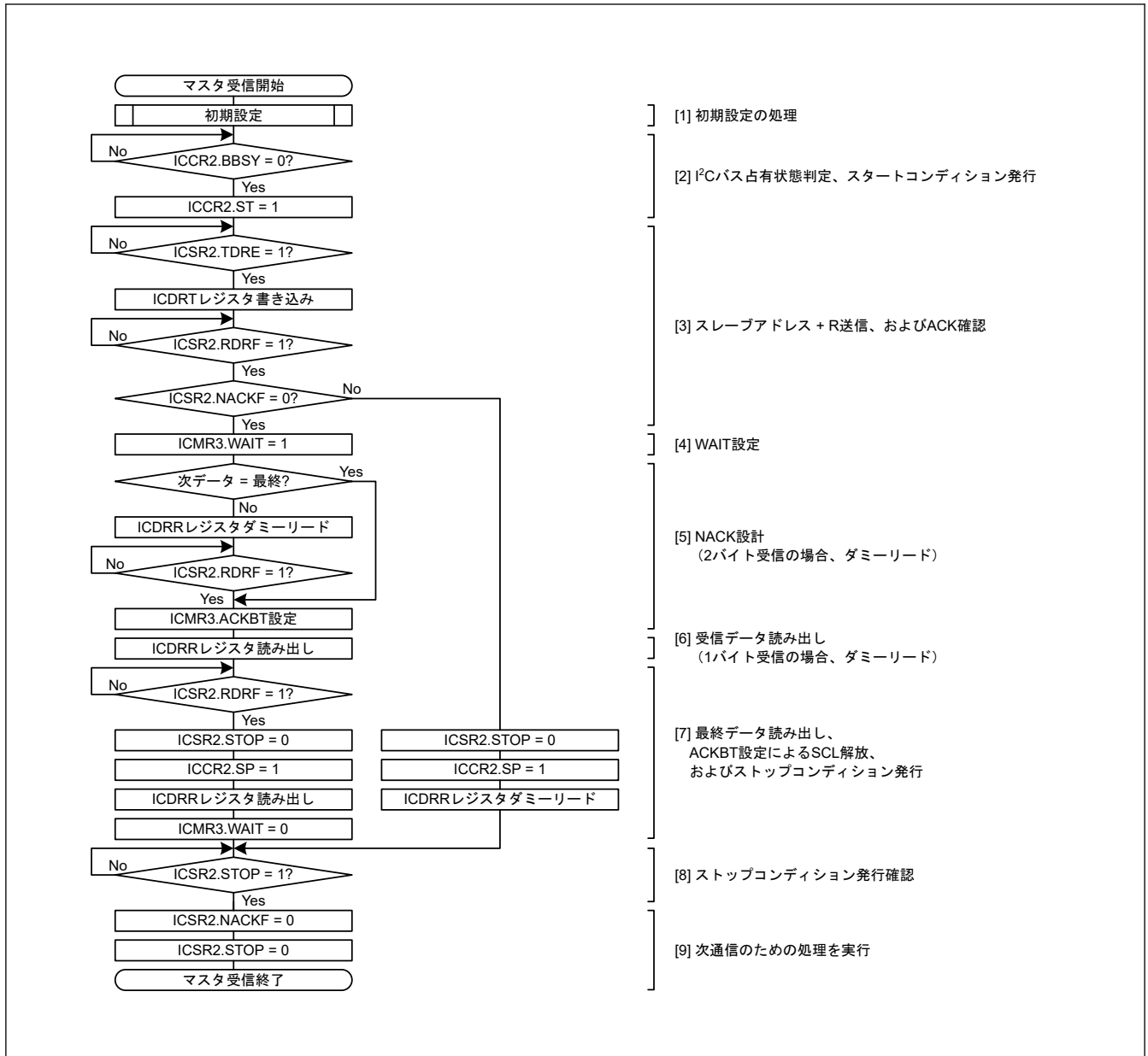
図 26.10 マスタ受信の例 (7ビットアドレスフォーマットで1または2バイト受信の場合)
