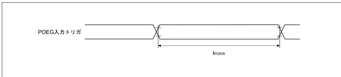
図 41.15 POEG 入カトリガタイミング
