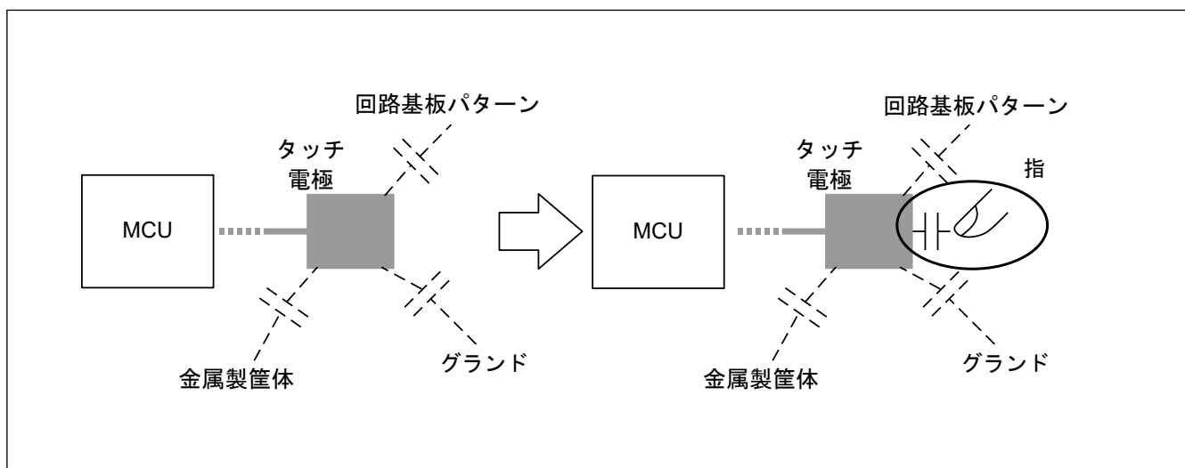
図 34.1 指による静電容量の増加
