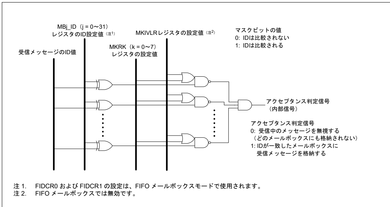
図 27.17 アクセプタンスフィルタ処理
