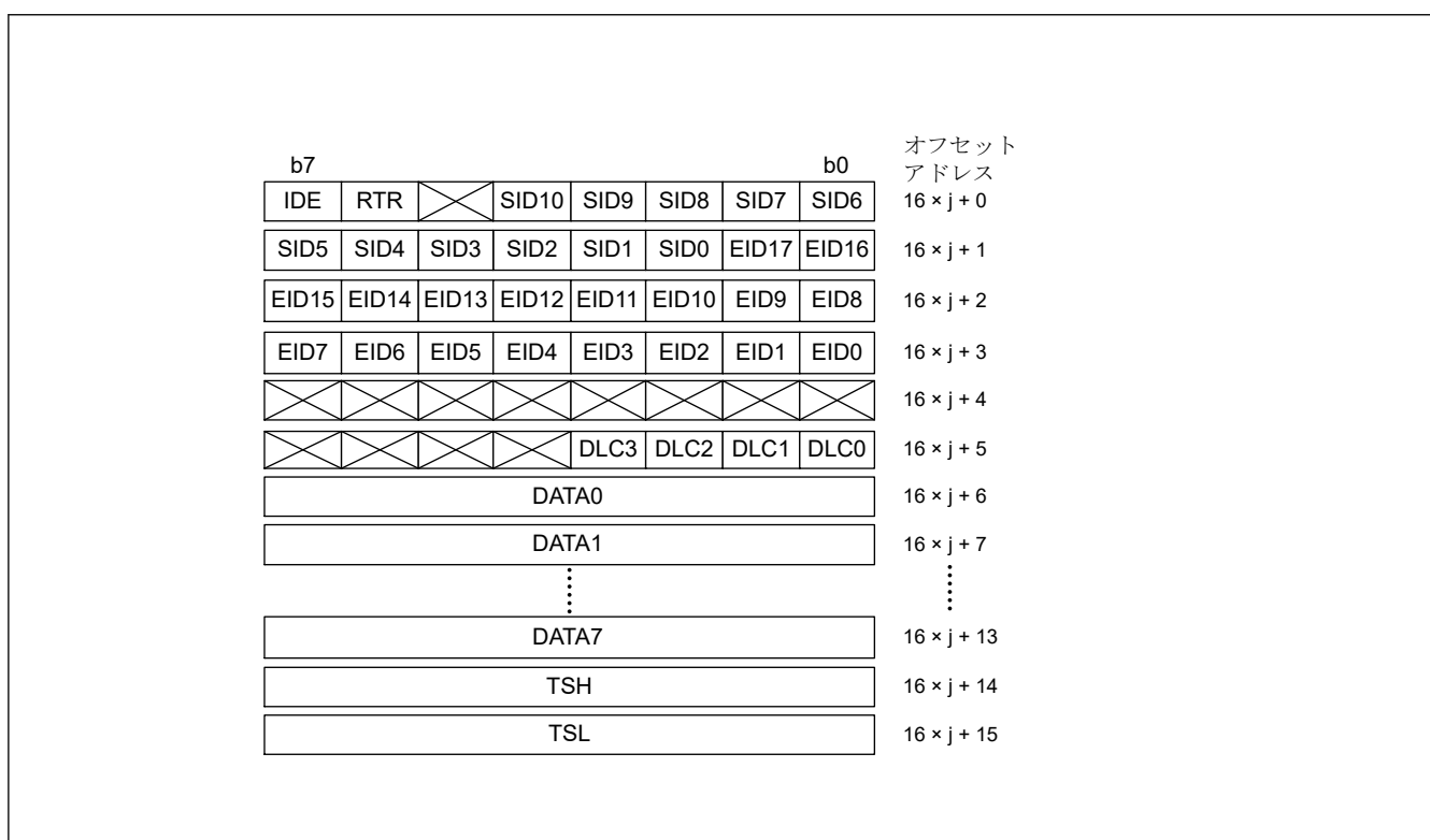
図 27.13 メールボックスレジスタの構造 (j = 0~31)
