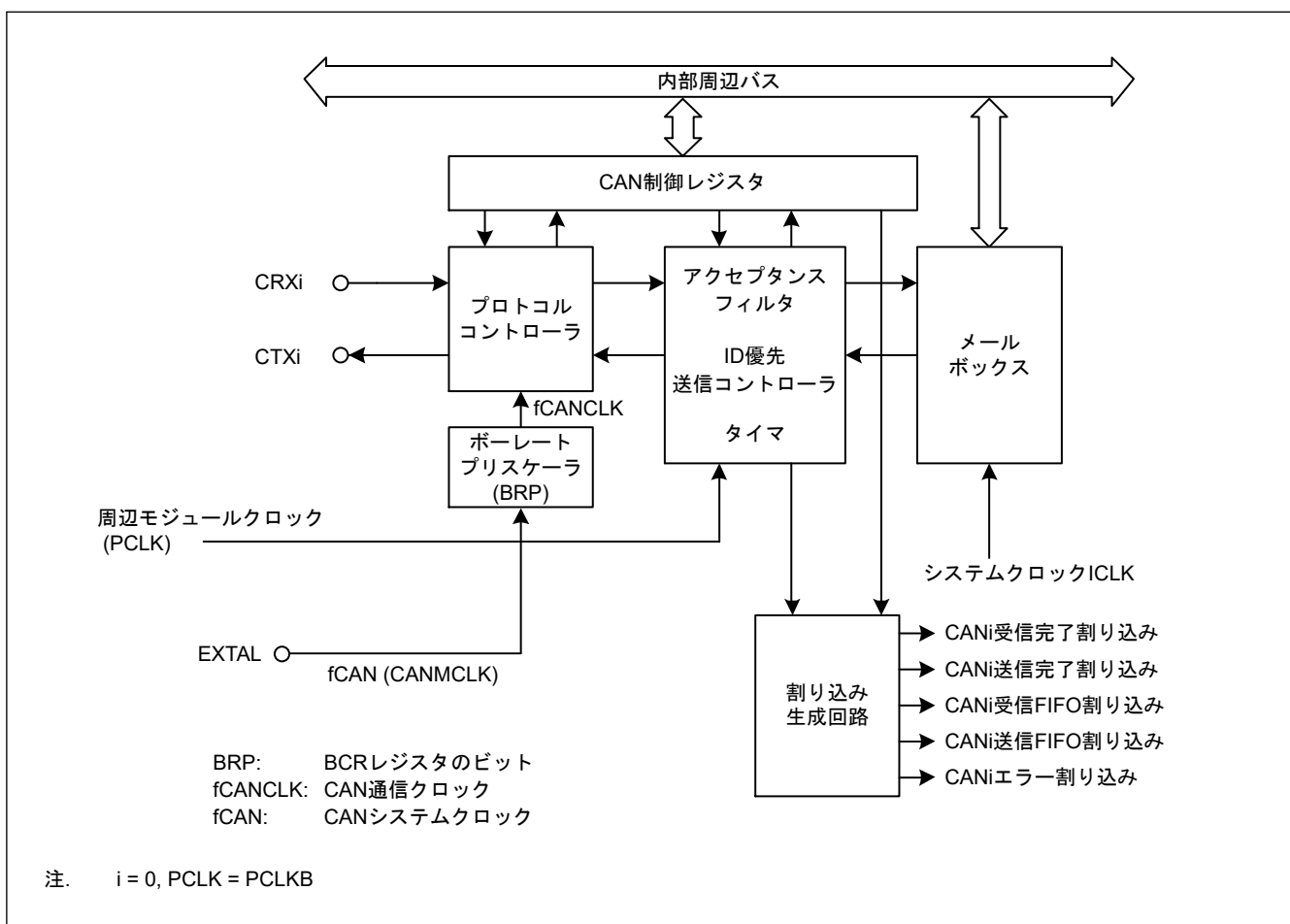
図 27.1 CAN モジュールブロック図
