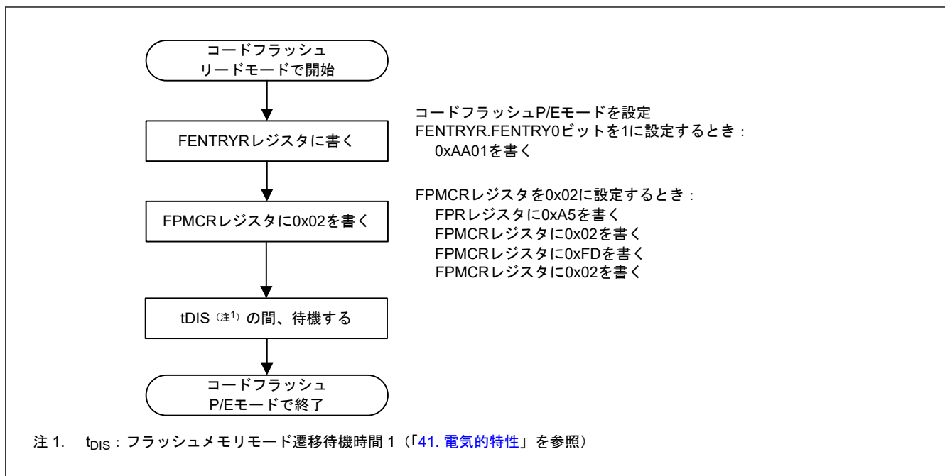
図 37.15 読み出しモードからコードフラッシュ P/E モードへの変更手順
