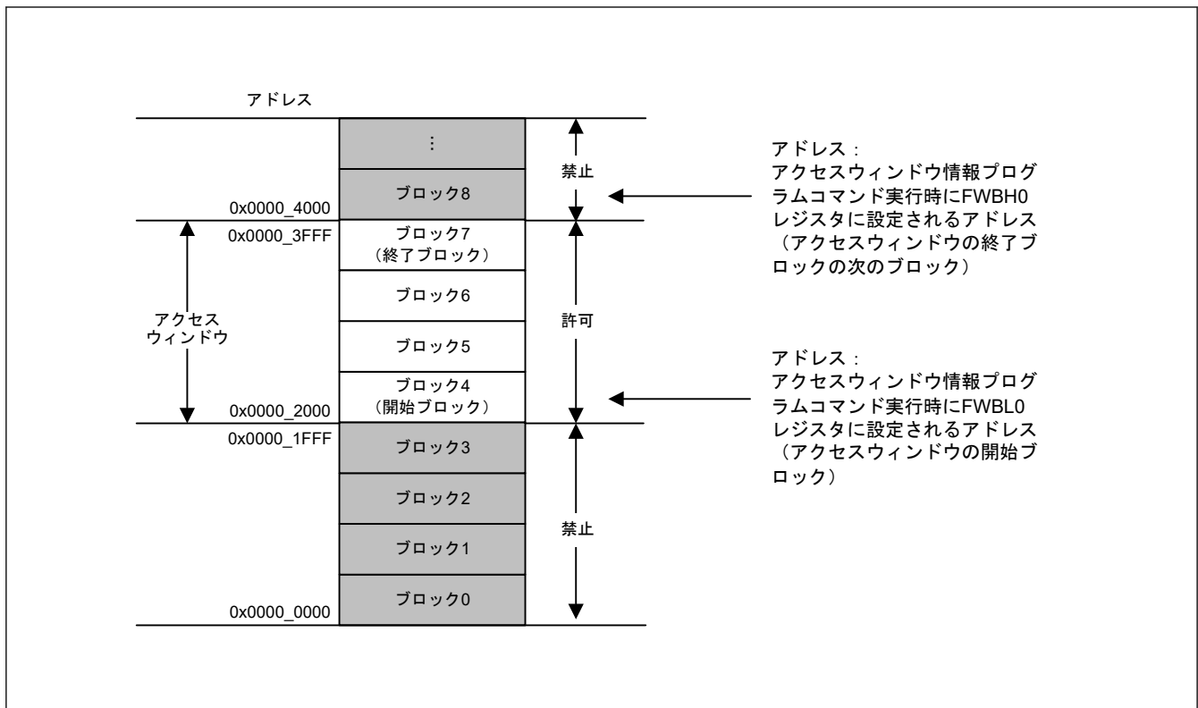
図 37.9 領域プロテクションの概要
