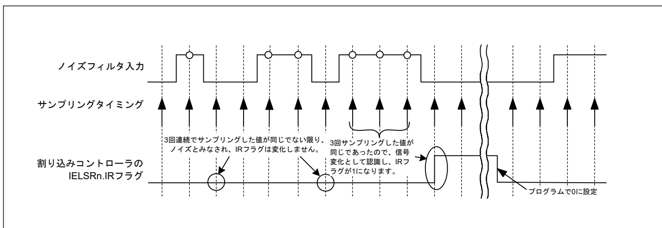
図 33.6 ノイズフィルタおよび割り込み動作例
