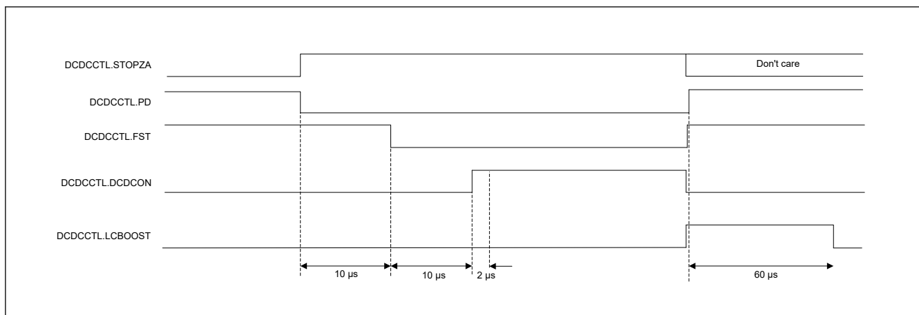
図 10.3 LDO 電源モード、DCDC 電源モード、Subosc-speed モード、ソフトウェアスタンバイモード間切り替え時の遷移タイミングとロード制限
