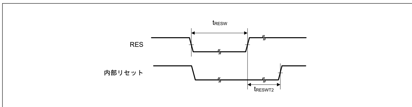
図 41.8 リセット入カタイミング (1)
