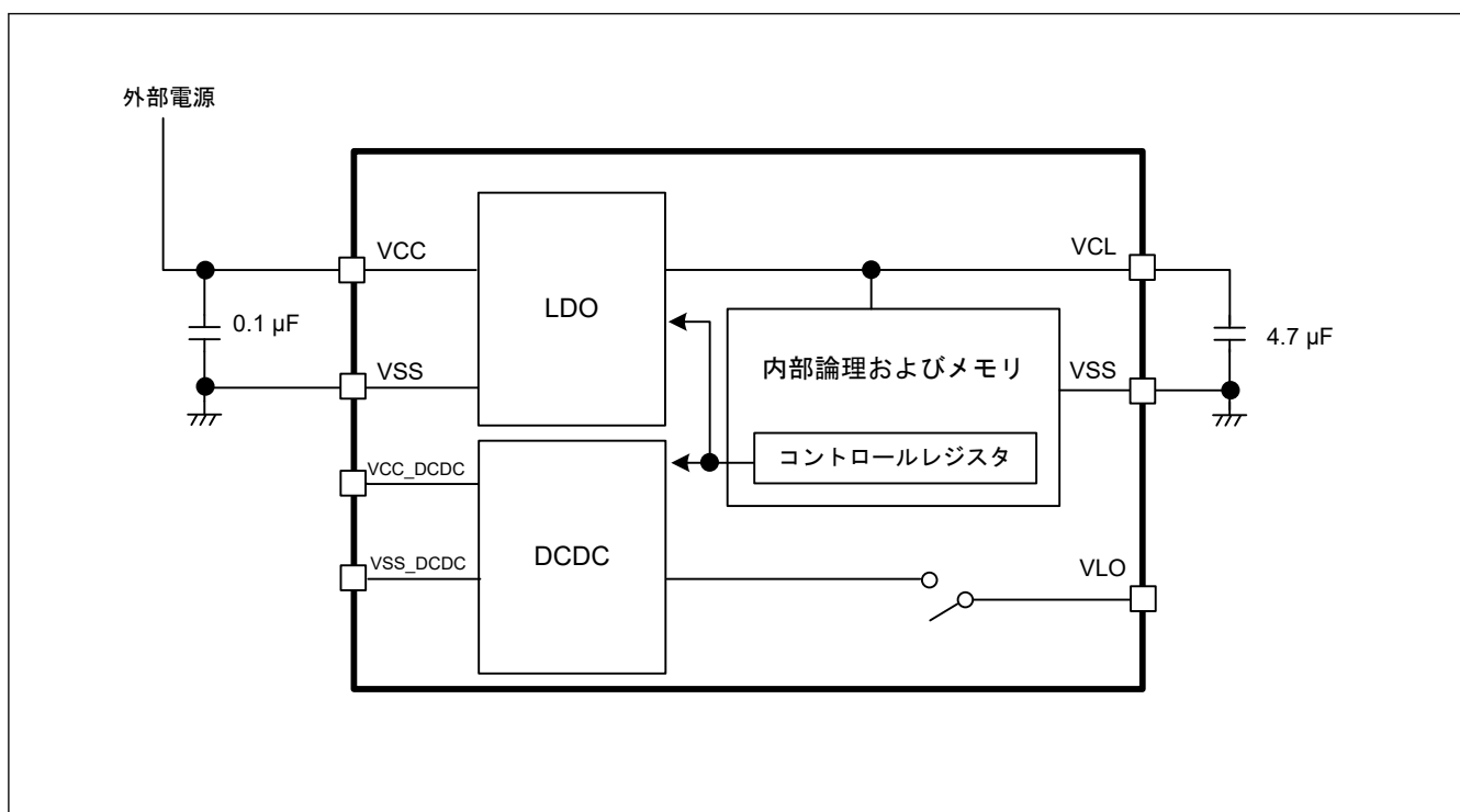
図 40.1 LDO の設定
