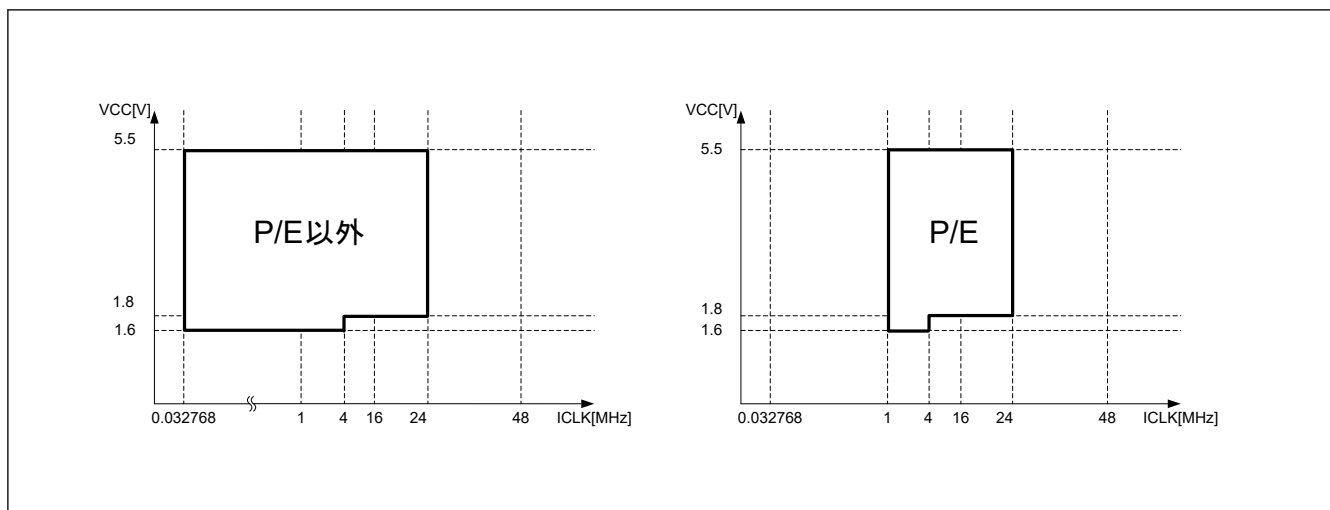
図 10.5 Middle-speed モードにおける動作電圧と動作周波数
