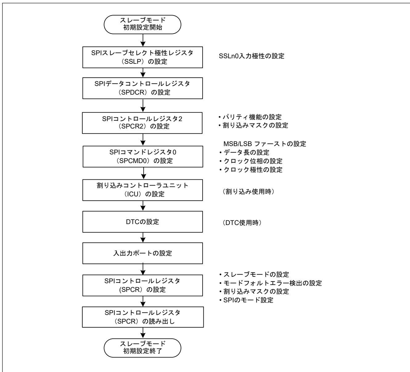
図 28.36 スレーブモード時の SPI 動作の初期化フロー例
