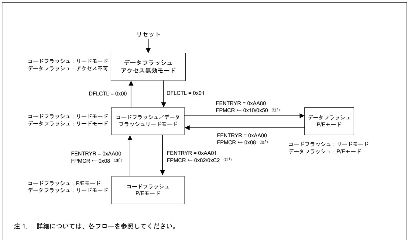
図 37.13 フラッシュメモリのモード遷移
