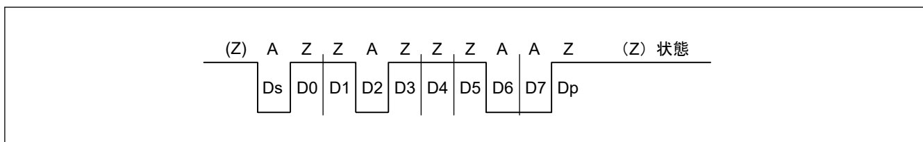
図 25.49 ダイレクトコンベンション (SCMR.SDIR ビット = 0、SCMR.SINV ビット = 0、SMR_SMCI.PM ビット = 0)
