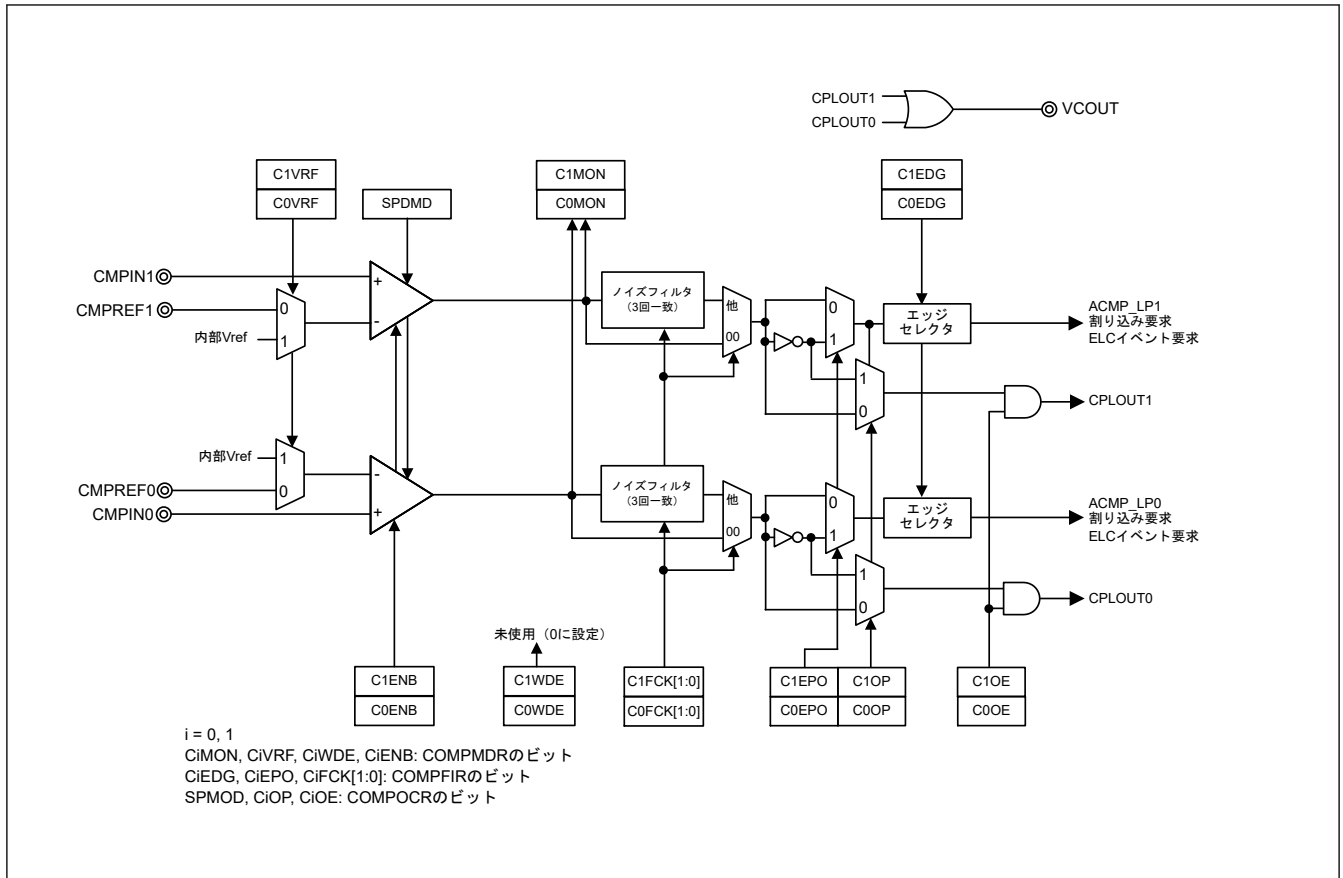
図 33.1 ウィンドウ機能無効時の ACMPLP ブロック図
