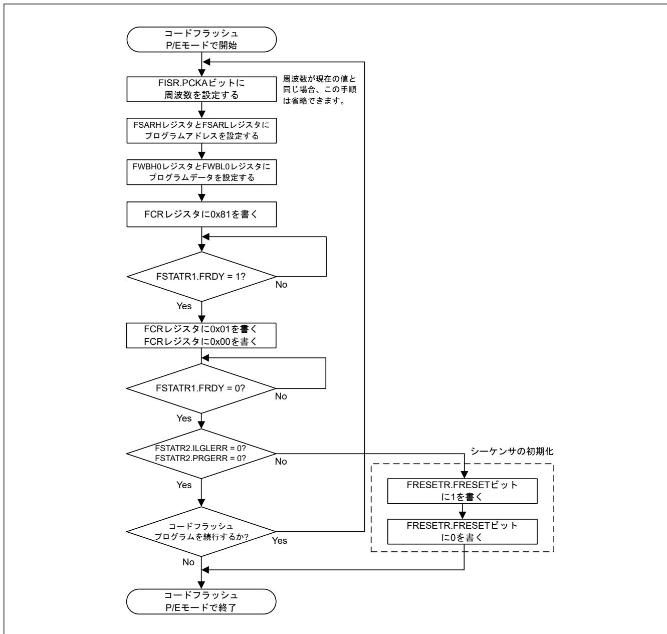
図 37.19 コードフラッシュのプログラム時のフローチャート
