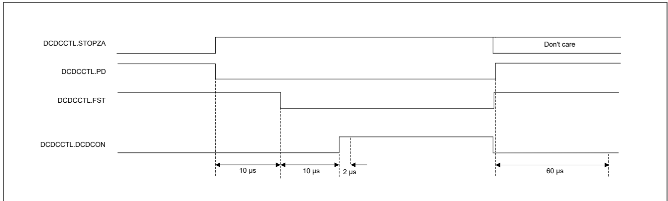
図 10.2 LDO 電源モードと DCDC 電源モード間切り替え時の遷移タイミングとロード制限
