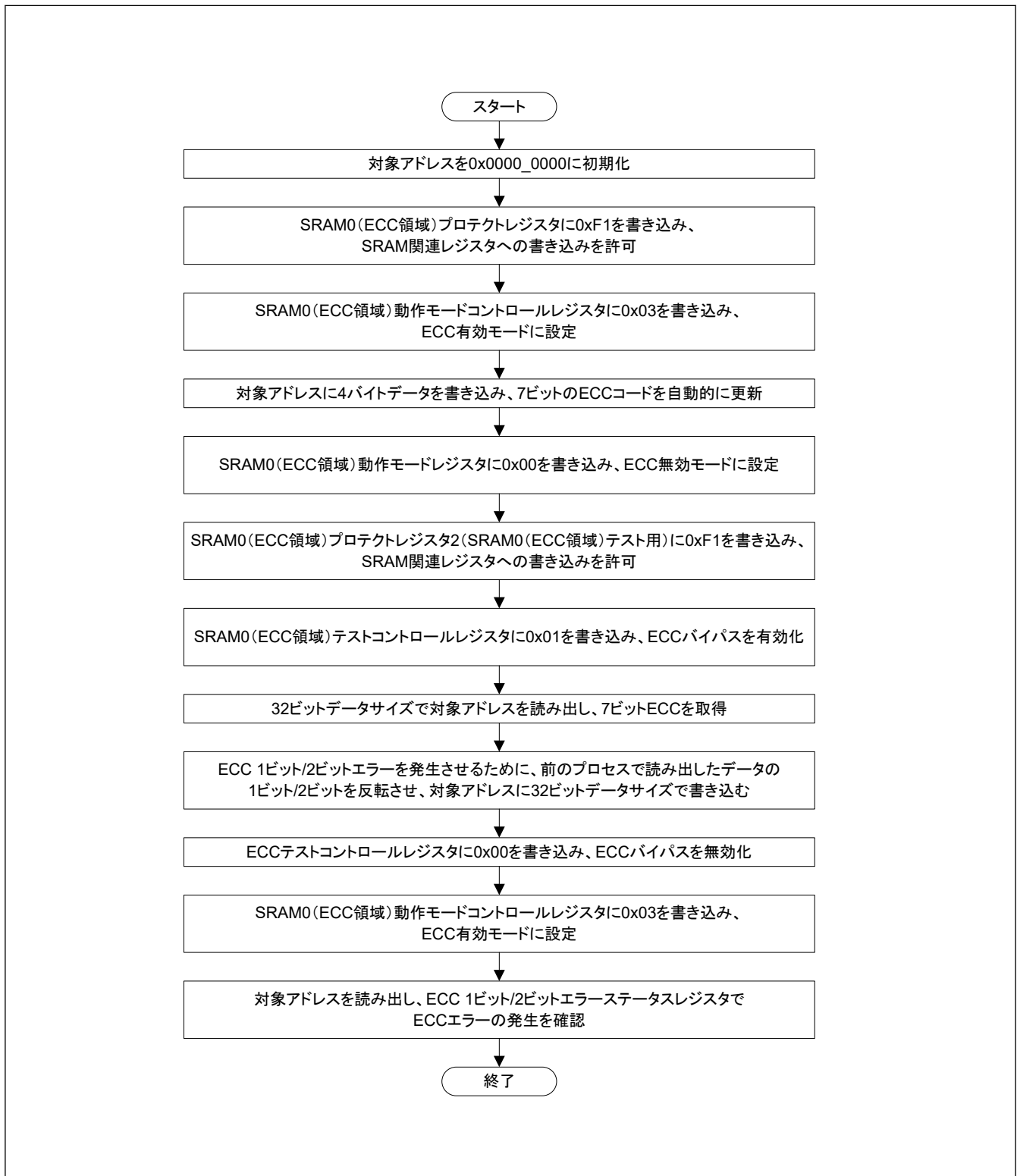
図 36.1 ECC デコーダのテスト方法
