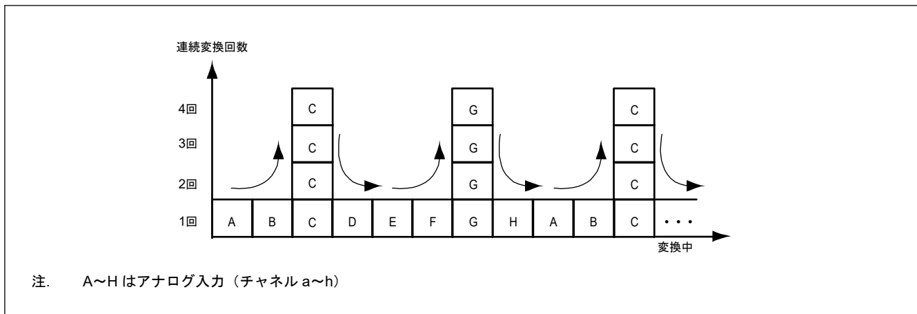
図 30.2 ADADC.ADC[2:0] = 011b および ADADS0/1 によるアナログ入力 C と G を 1 に選択時のスキャン変換シーケンス
