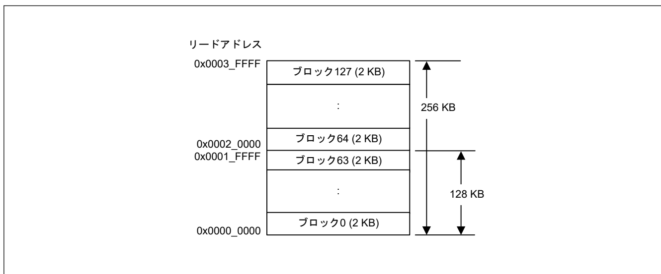
図 37.2 コードフラッシュメモリマッピング
