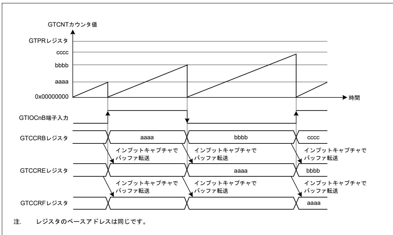
図 20.18 GTCRA および GTCCRB レジスタのダブルバッファ動作例 (GTIOcNB 端子入力の両エッジでインプットキャプチャ、のこぎり波でアップカウント、GTIOcNB 端子入力の両エッジで GTCNT カウンタクリアの場合)
