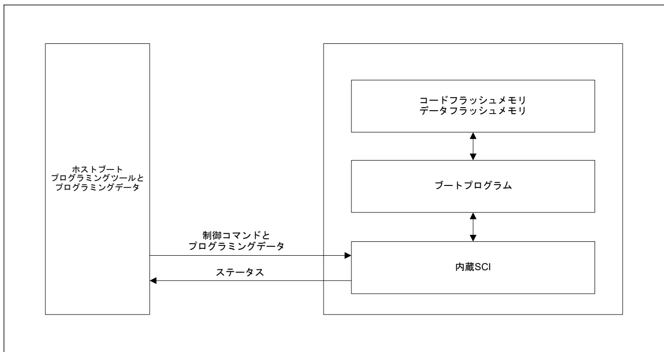
図 37.10 SCI ブートモード時のシステム構成
