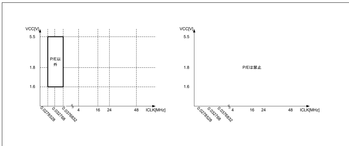
図 10.7 Subosc-speed モードにおける動作電圧と動作周波数
