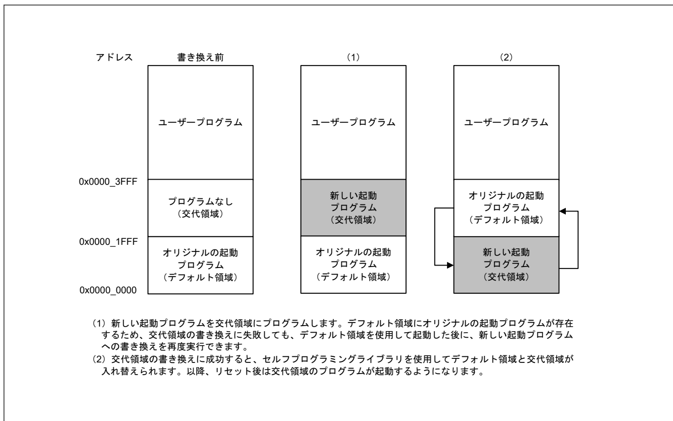
図 37.6 スタートアッププログラムプロテクションの概要
