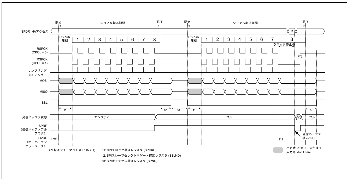
図 28.29 マスタモードの受信バッファフル状態でシリアル転送が継続するときのクロック停止波形 (SPCMDm.CPHA = 1)
