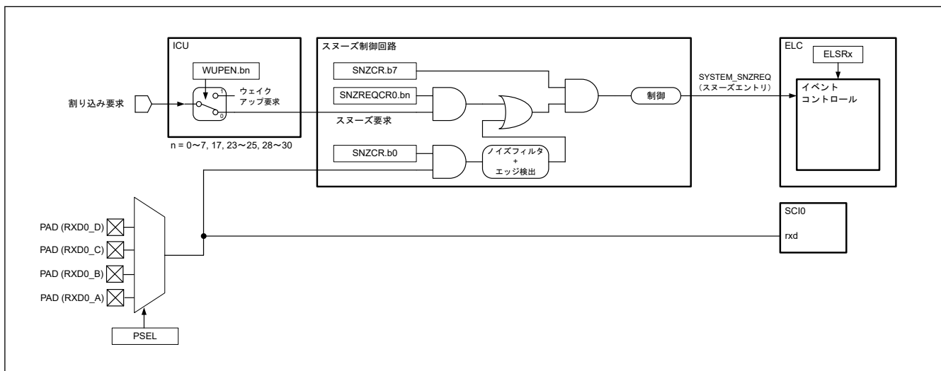
図 10.9 スヌーズモードエントリの構成
