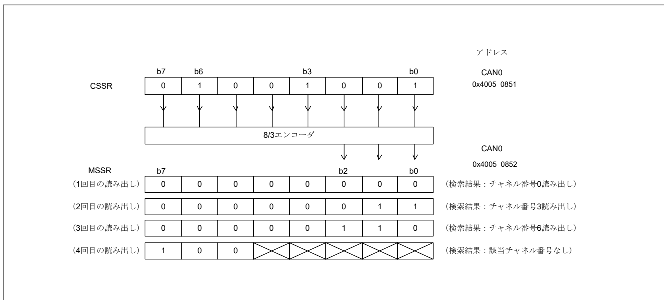
図 27.4 CSSR レジスタおよび MSSR レジスタの書き込みおよび読み出し動作
