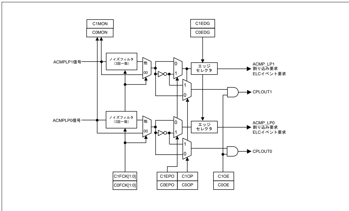
図 33.5 ノイズフィルタおよびエッジ検出の構成
