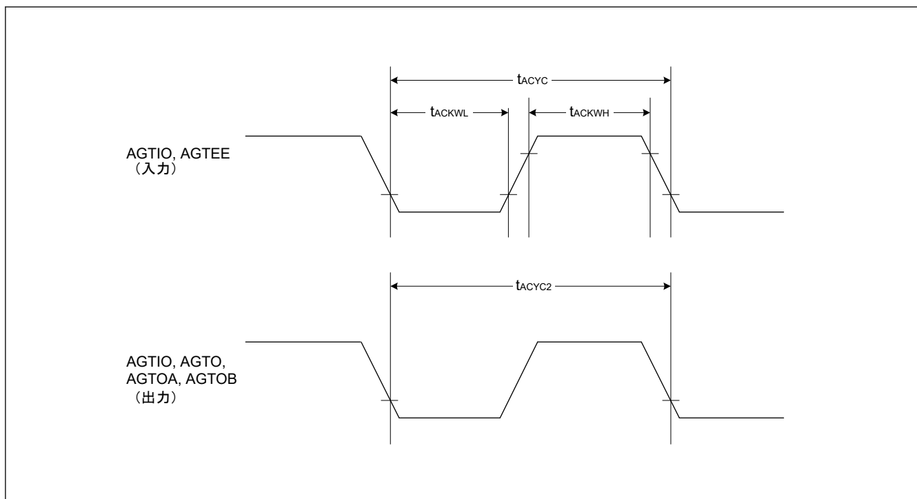
図 41.17 AGT 入出力タイミング
