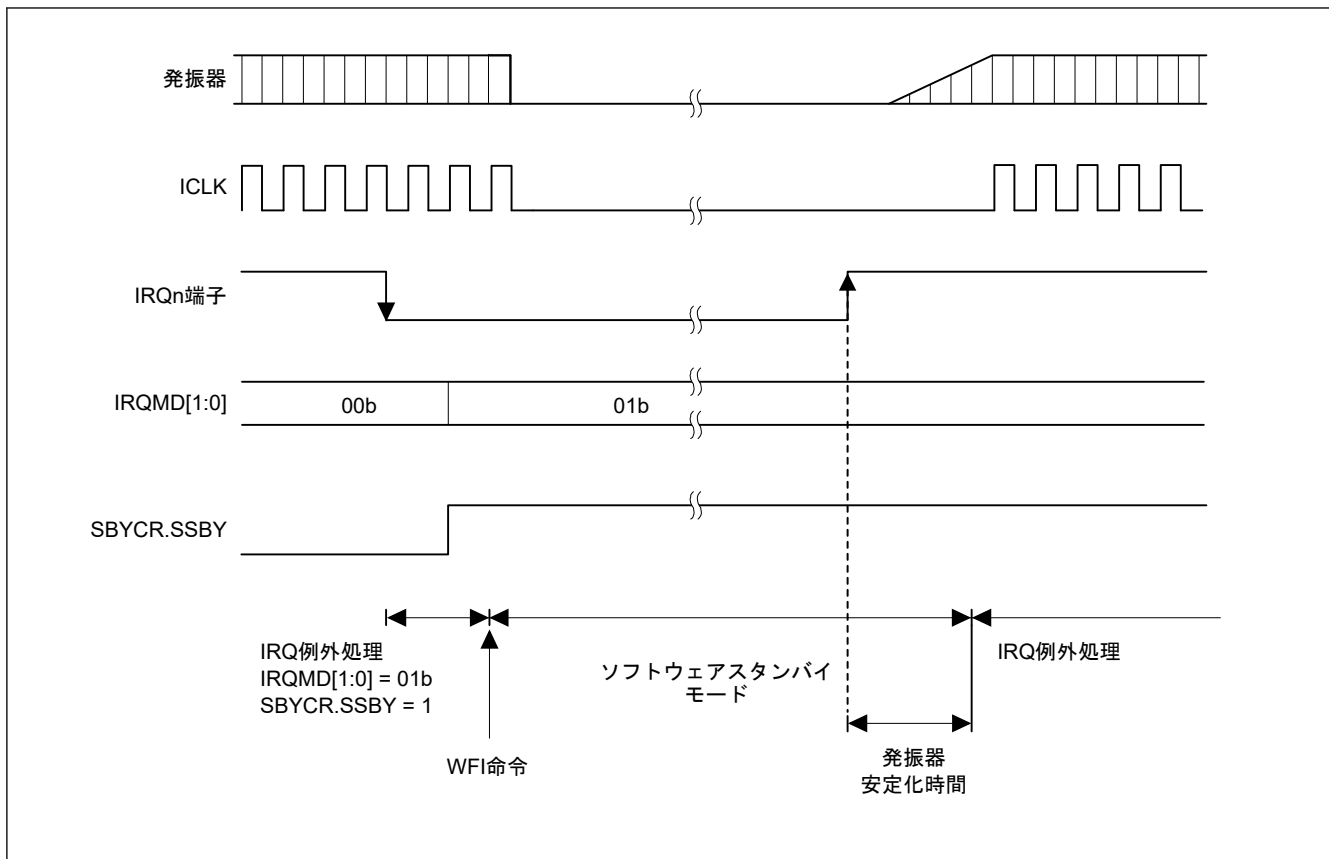
図 10.8 ソフトウェアスタンバイモードの応用例
