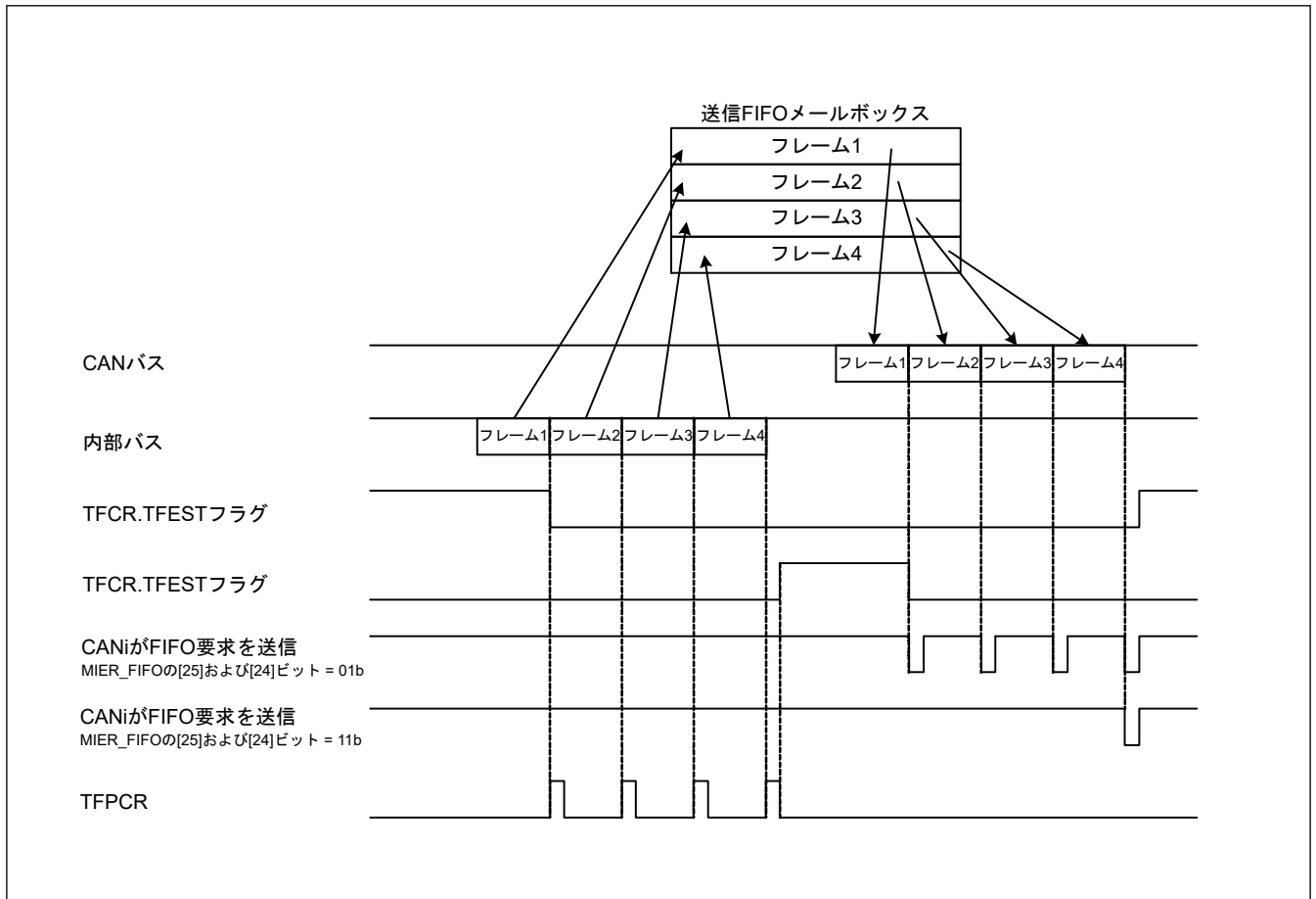
図 27.3 MIER_FIFO のビット[25]および[24]が 01b または 11b の場合の送信 FIFO メールボックスの動作説明
