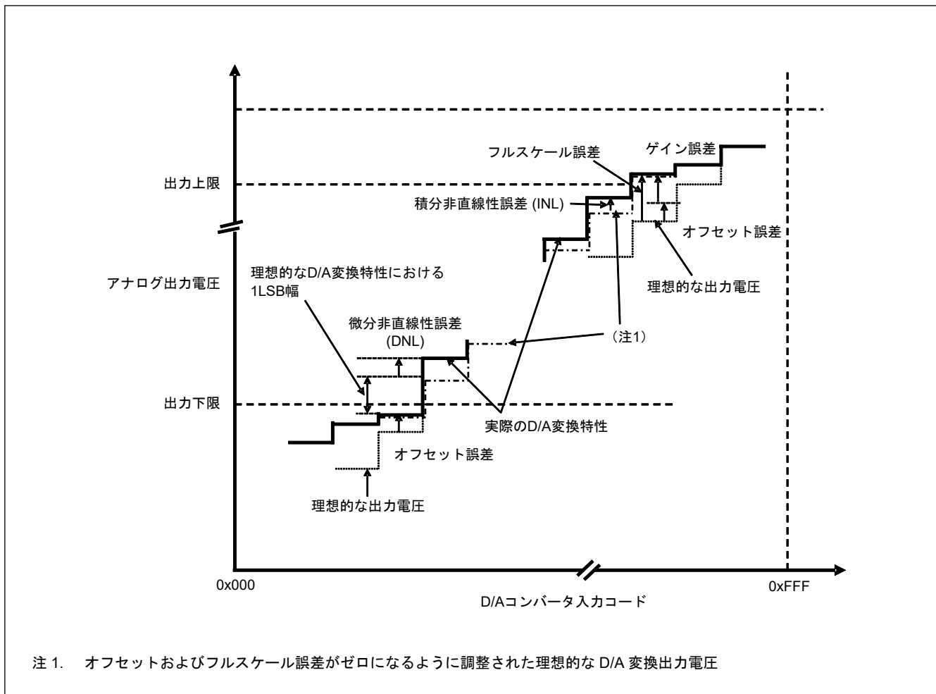
図 41.40 D/A コンバータ特性用語の解説図
