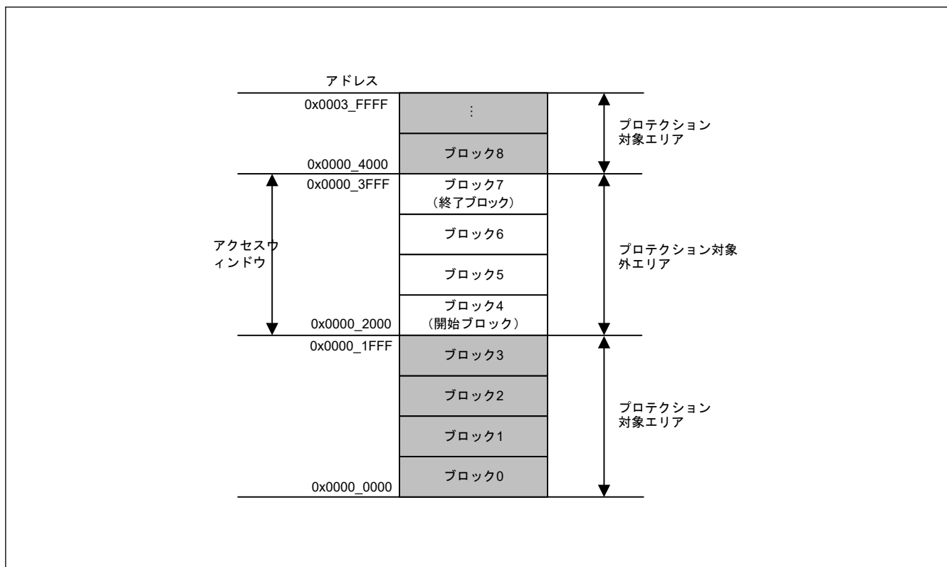
図 37.7 フラッシュ領域プロテクションの概要
