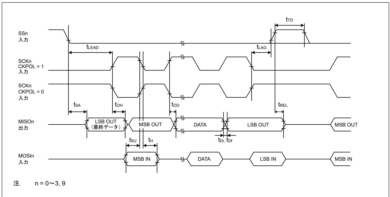
図 41.26 SCI 簡易 SPI モードタイミング (スレーブ、CKPH = 0)
