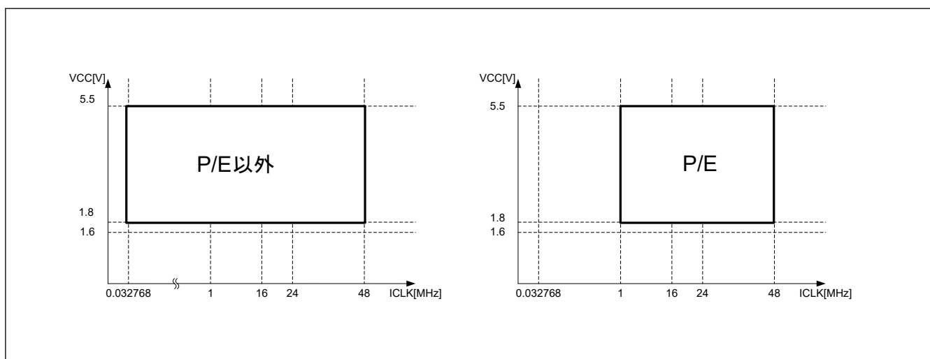
図 10.4 High-speed モードにおける動作電圧と動作周波数
