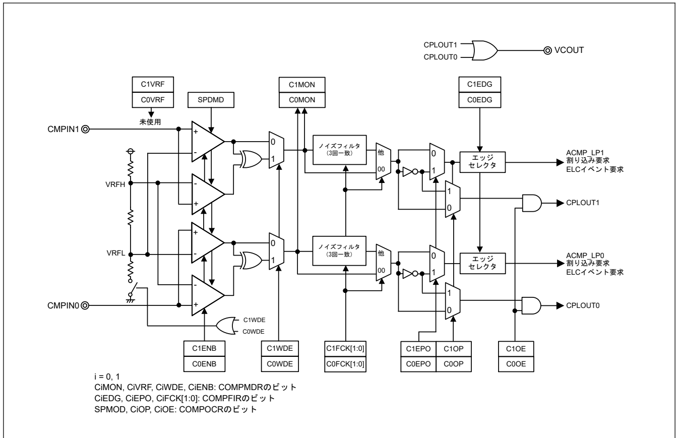
図 33.2 ウィンドウ機能有効時の ACMPLP ブロック図
