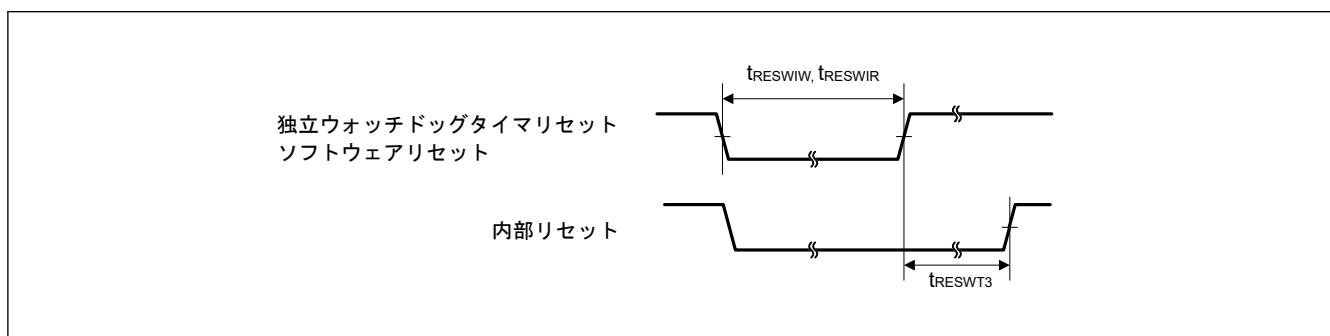
図 41.9 リセット入カタイミング (2)
