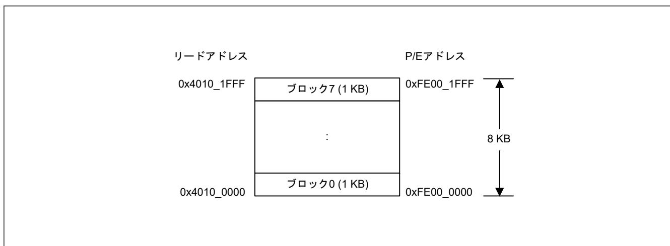
図 37.3 データフラッシュメモリマッピング
