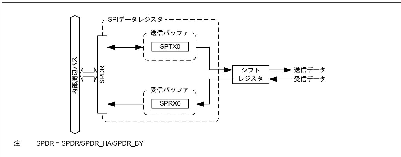
図 28.2 SPDR/SPDR_HA/SPDR_BY レジスタの構成図
