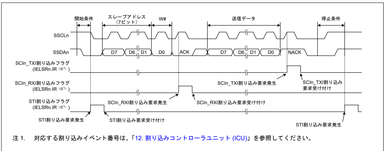
図 25.64 簡易 IIC モードにおけるマスタ送信の動作例 2 (7 ビットスレーブアドレス、ACK 割り込み、NACK 割り込み使用時)
