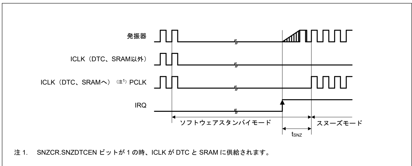
図 41.11 ソフトウェアスタンバイモードからスヌーズモードへの復帰タイミング
