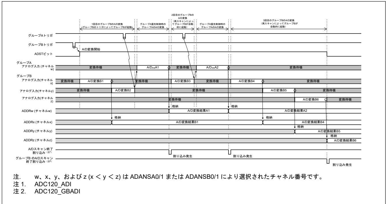
図 30.18 グループ優先動作の例 1-2 : グループ B 再スキャン中のグループ A トリガ入力、再スキャンあり (ADGSPCR.GBRSCN = 1、ADGSPCR.GBRP = 0 の場合)
