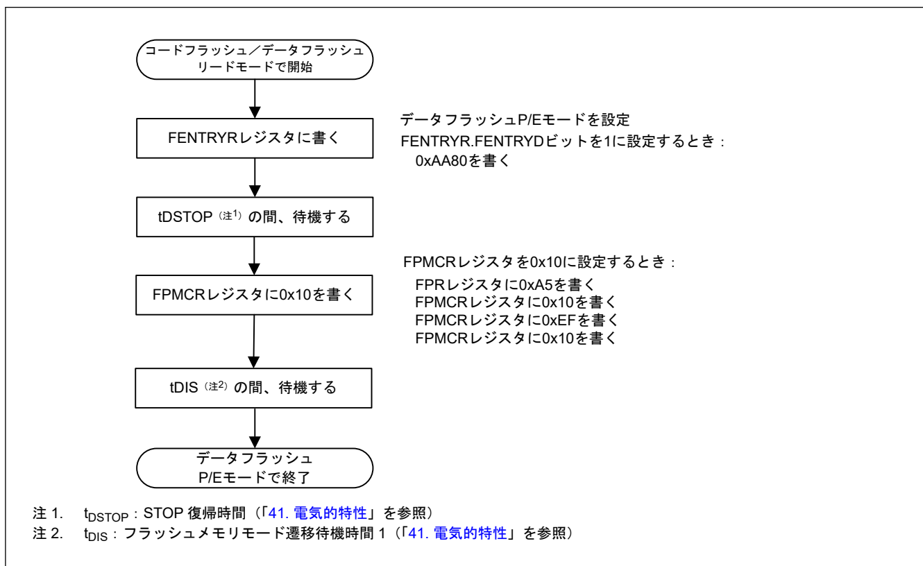
図 37.16 読み出しモードからデータフラッシュ P/E モードへの変更手順
