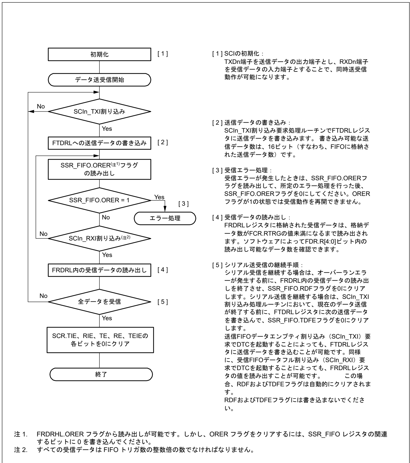
図 25.46 クロック同期式モードにおけるシリアル同時送受信動作のフローチャート例 (FIFO 選択時)
