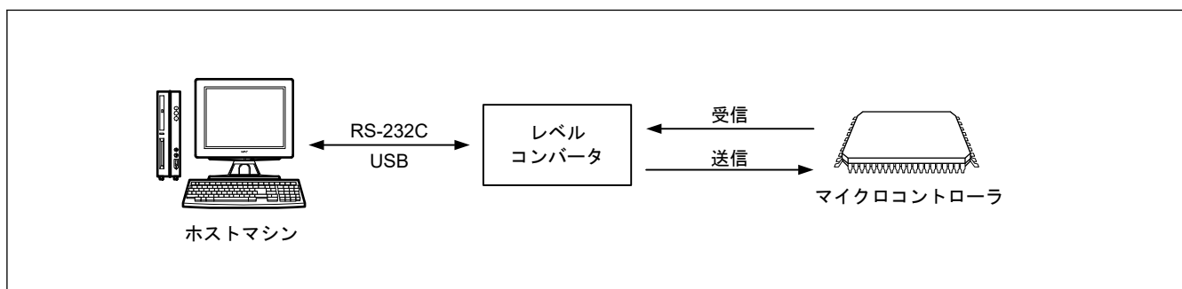
図 37.11 フラッシュメモリにプログラムを書き込むための環境
