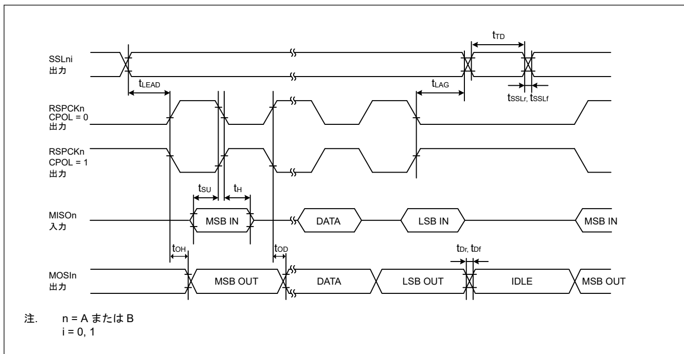
図 41.31 SPI タイミング (マスタ、CPHA = 1) (ビットレート : PCLKA を 2 分周以外に設定)
