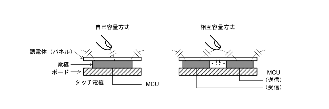
図 34.2 自己容量方式と相互容量方式
