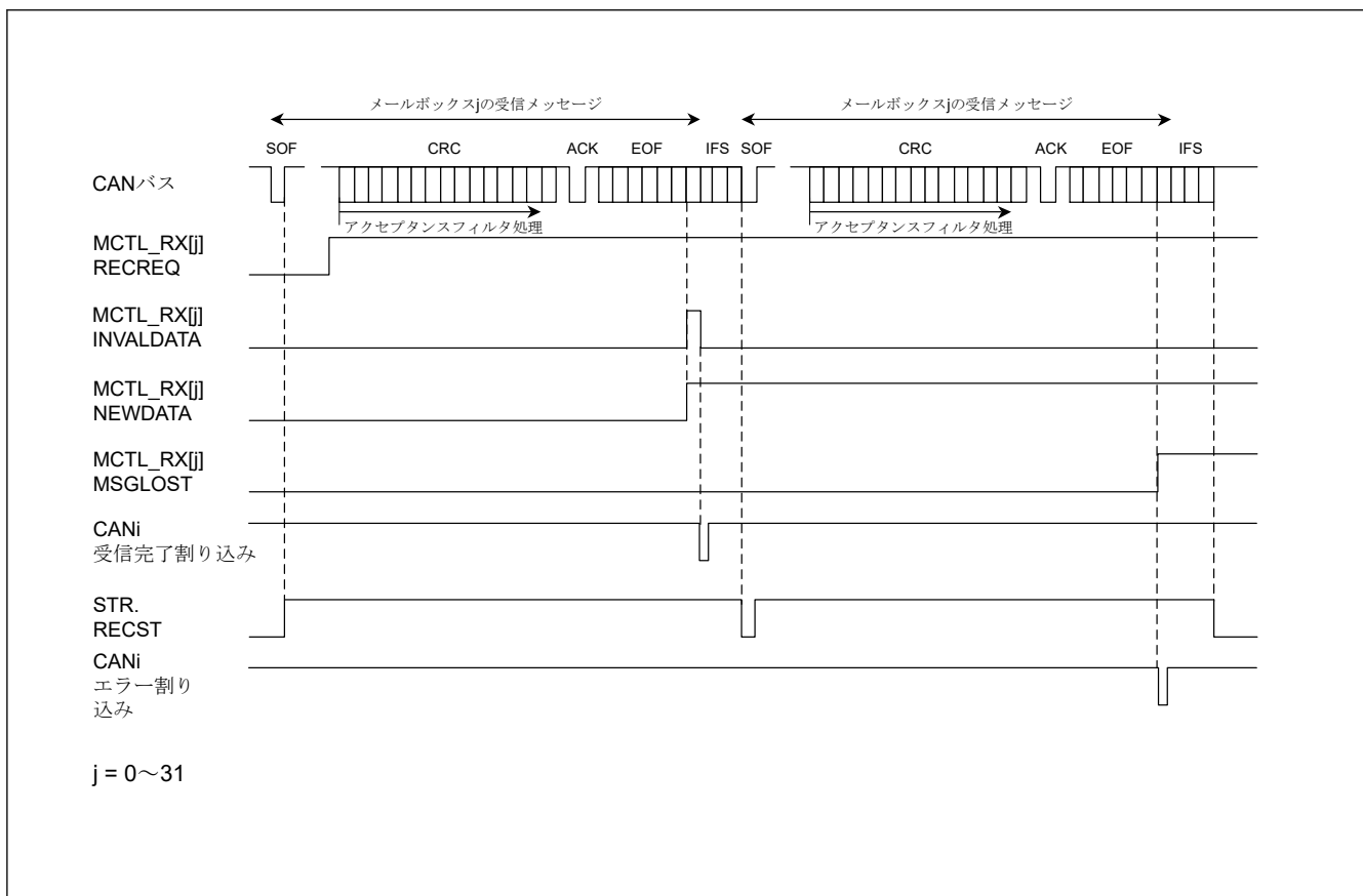
図 27.19 オーバーランモードでのデータフレーム受信の動作例
