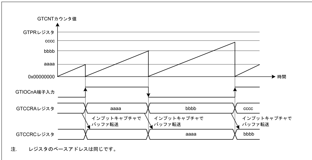
図 20.17 GTCRA および GTCCRB レジスタのバッファ動作例 (GTIOcNA 端子入力の両エッジでインプットキャプチャ、のこぎり波でアップカウント、GTIOcNA 端子入力の両エッジで GTCNT カウンタクリアの場合)
