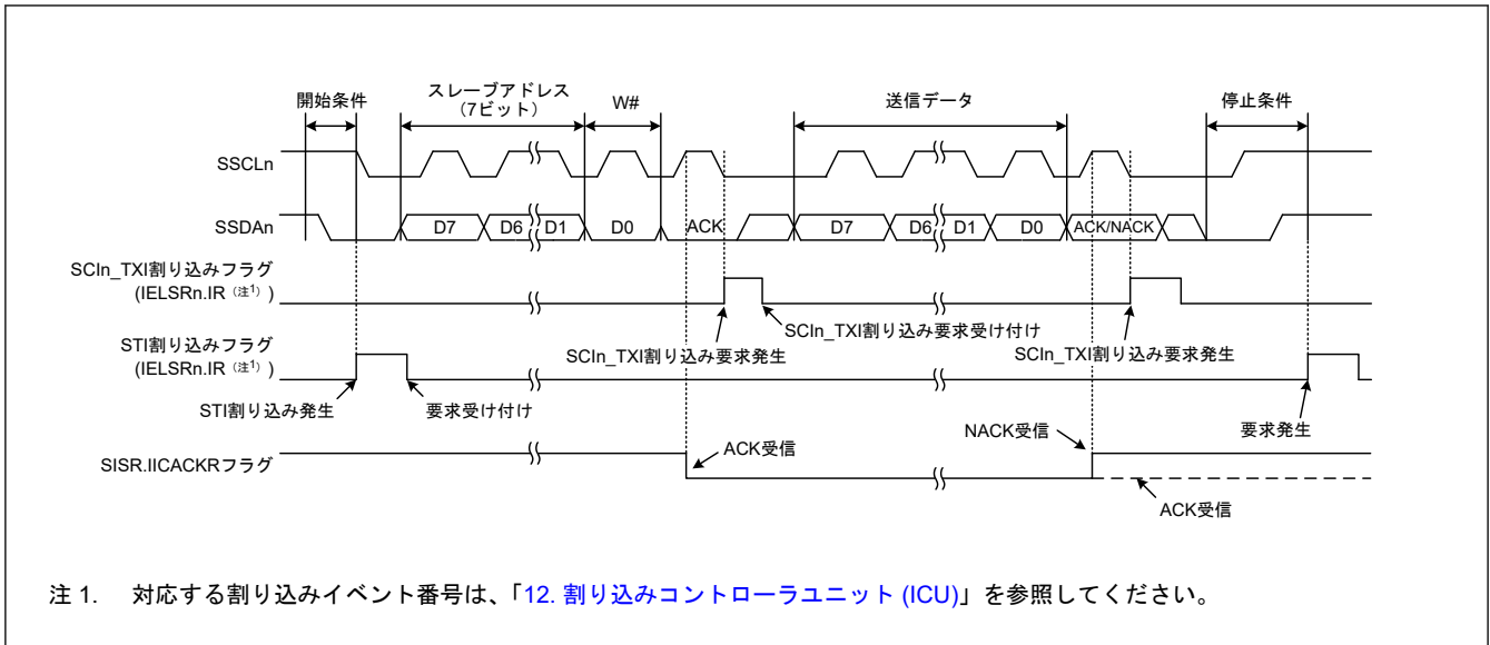
図 25.63 簡易 IIC モードにおけるマスタ送信の動作例 1 (7 ビットスレーブアドレス、送信割り込み、受信割り込み使用時)
