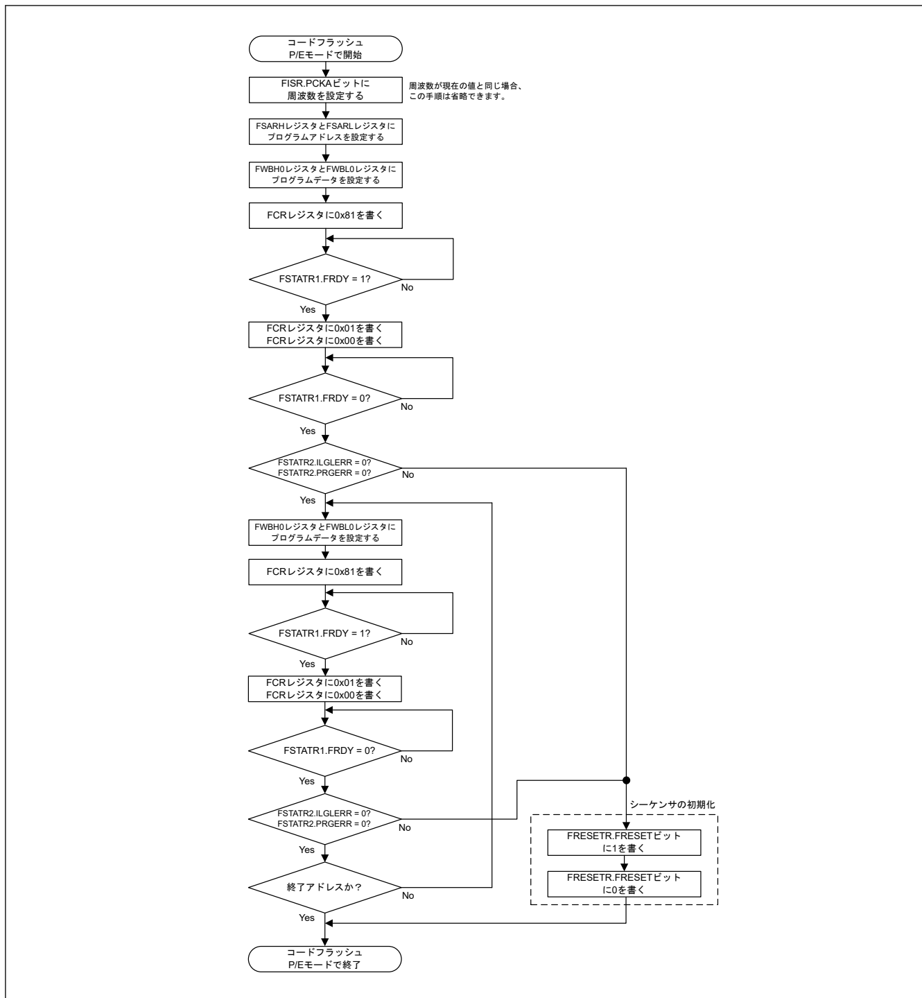
図 37.21 コードフラッシュの連続プログラム時のフローチャート
