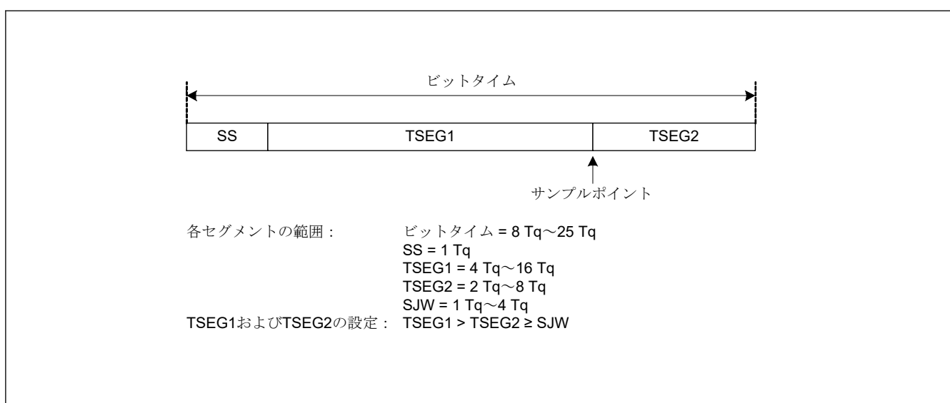
図 27.12 ビットタイミング
