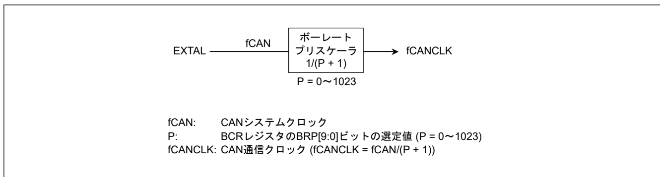
図 27.11 CAN クロック発振器のブロック図
