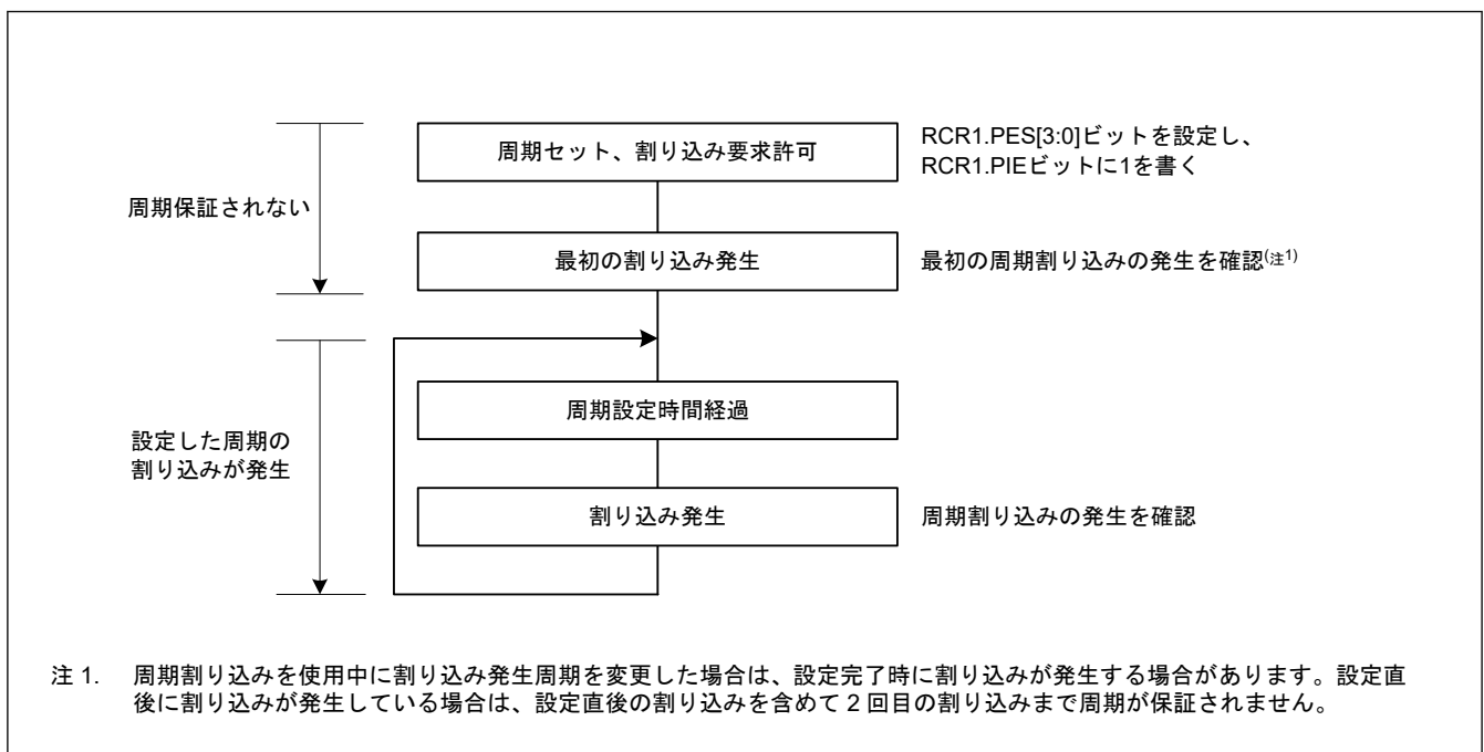
図 22.11 周期割り込み機能の使用法
