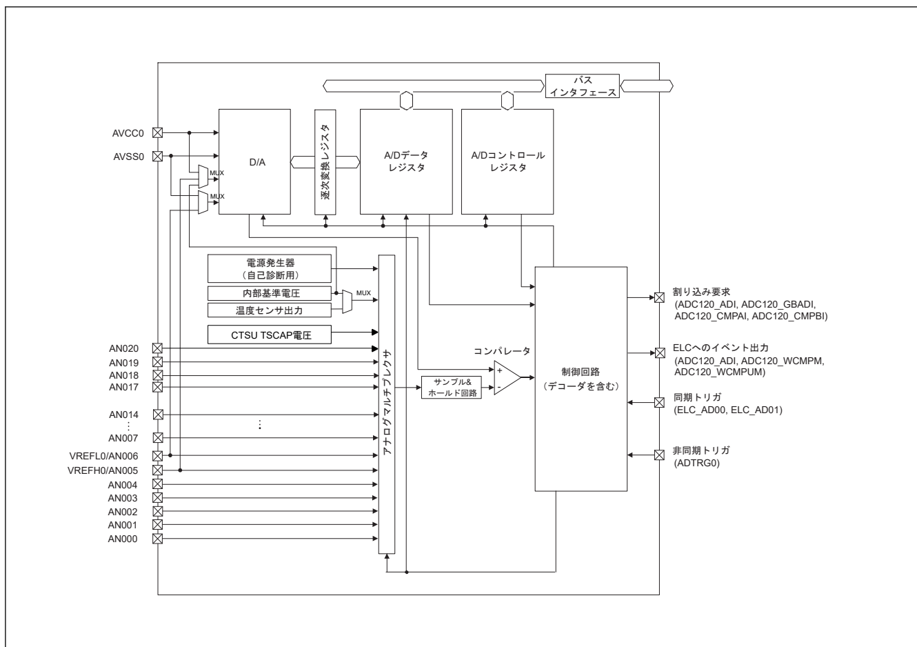
図 30.1 ADC12 のブロック図
