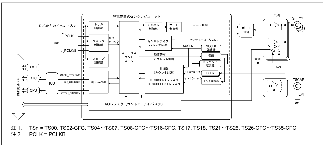
図 34.3 CTSU ブロック図
