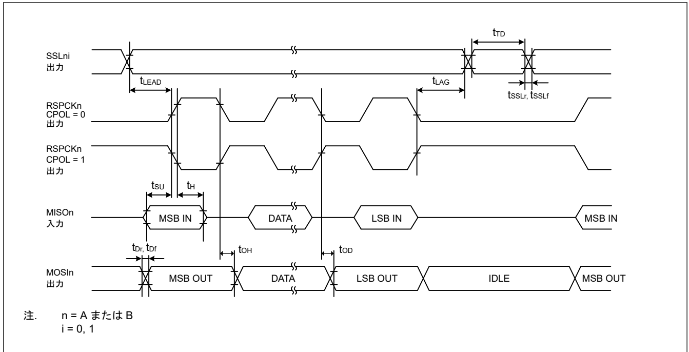
図 41.29 SPI タイミング (マスタ、CPHA = 0) (ビットレート : PCLKA を 2 分周以外に設定)
