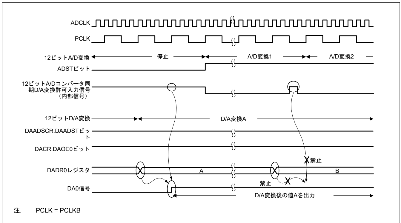
図 31.4 DAC12 が次からの同期 D/A 変換許可入力信号を取り込めない場合の例：ADC12
