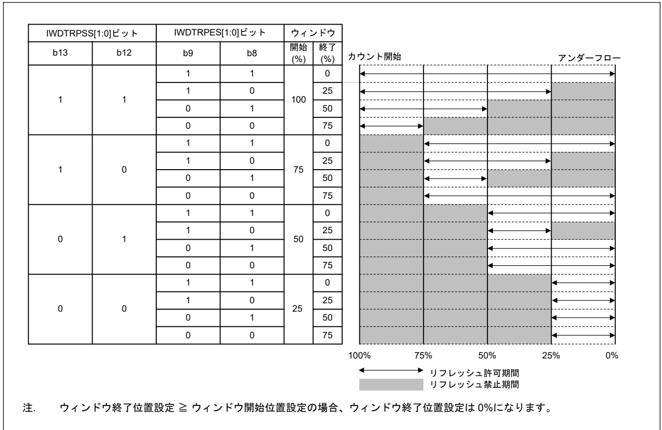
図 24.2 IWDRPSS[1:0]および IWDTRPES[1:0]ビットとリフレッシュ許可期間
