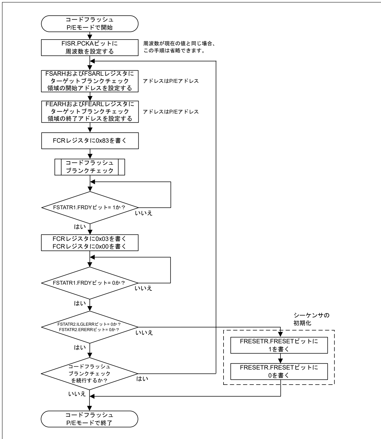
図 37.27 コードフラッシュブランクチェック手順のフローチャート
