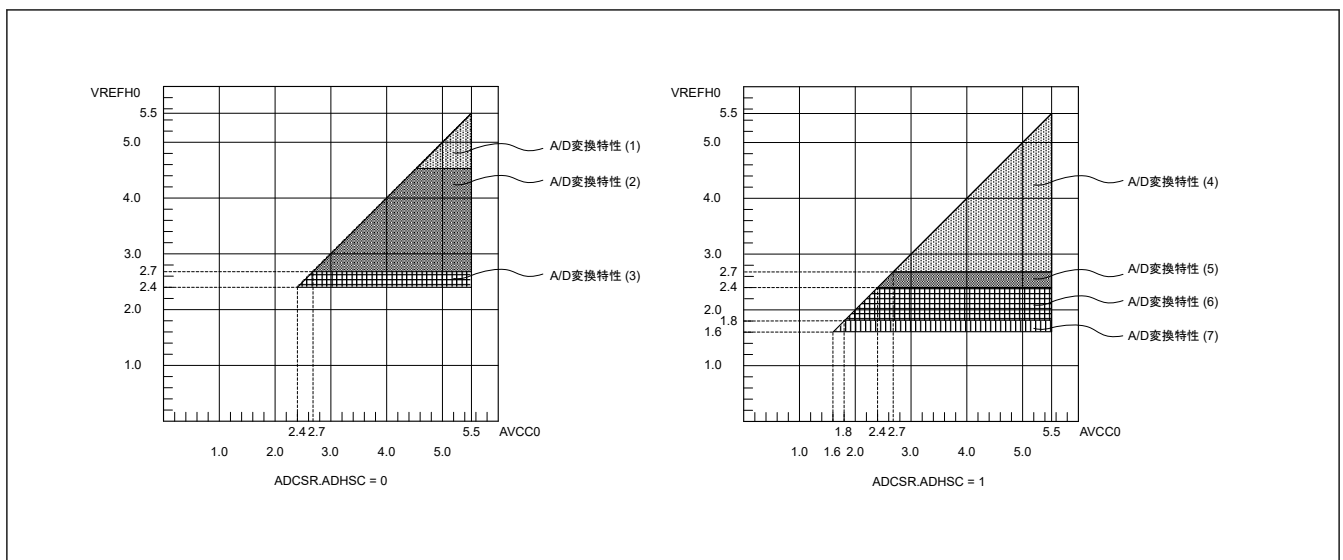
図 41.37 AVCC0~VREFH0 電圧範囲
