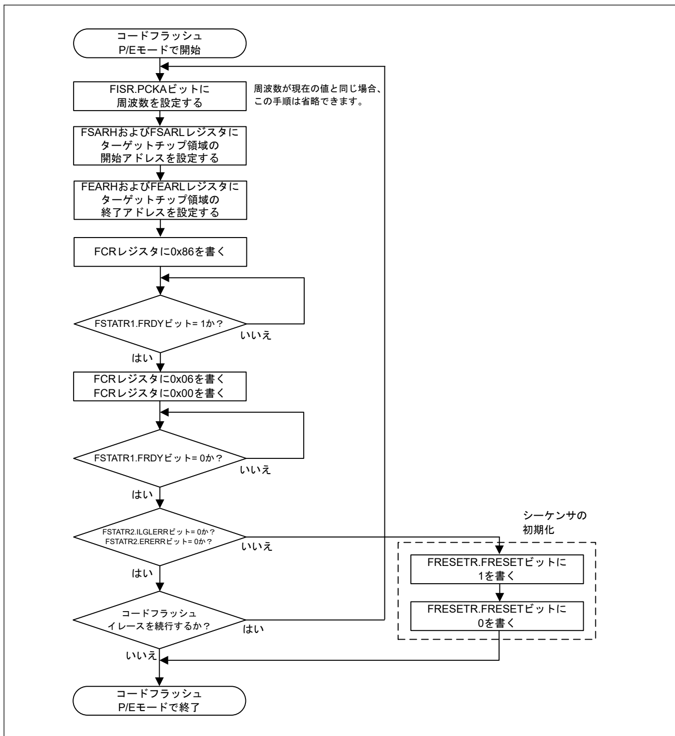
図 37.25 コードフラッシュチップイレース手順のフローチャート
