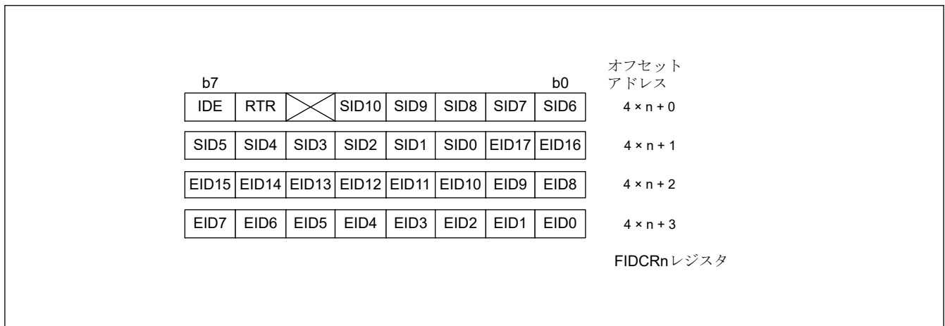
図 27.15 FIDCRn レジスタの構造 (n = 0)
