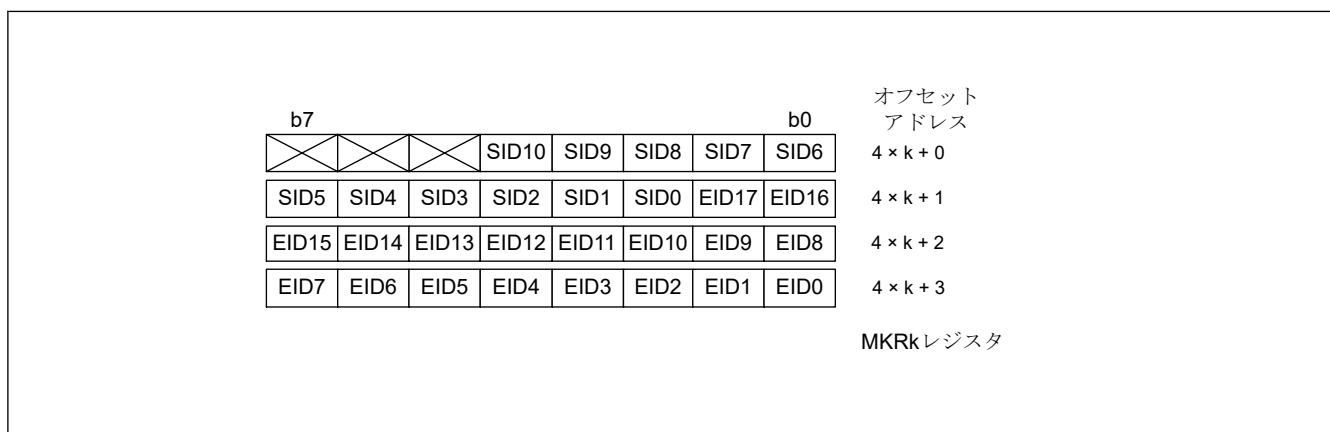
図 27.14 マスクレジスタの構造 (j = 0~7)
