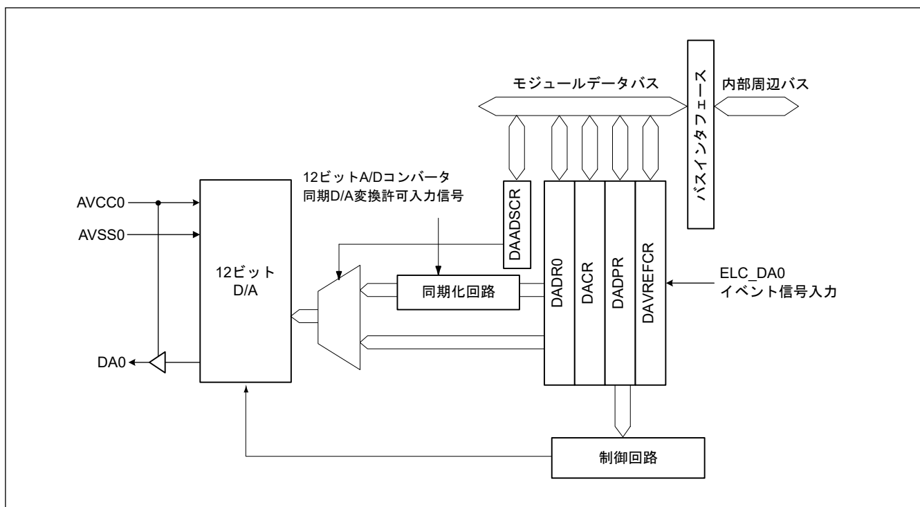
図 31.1 DAC12 のブロック図
