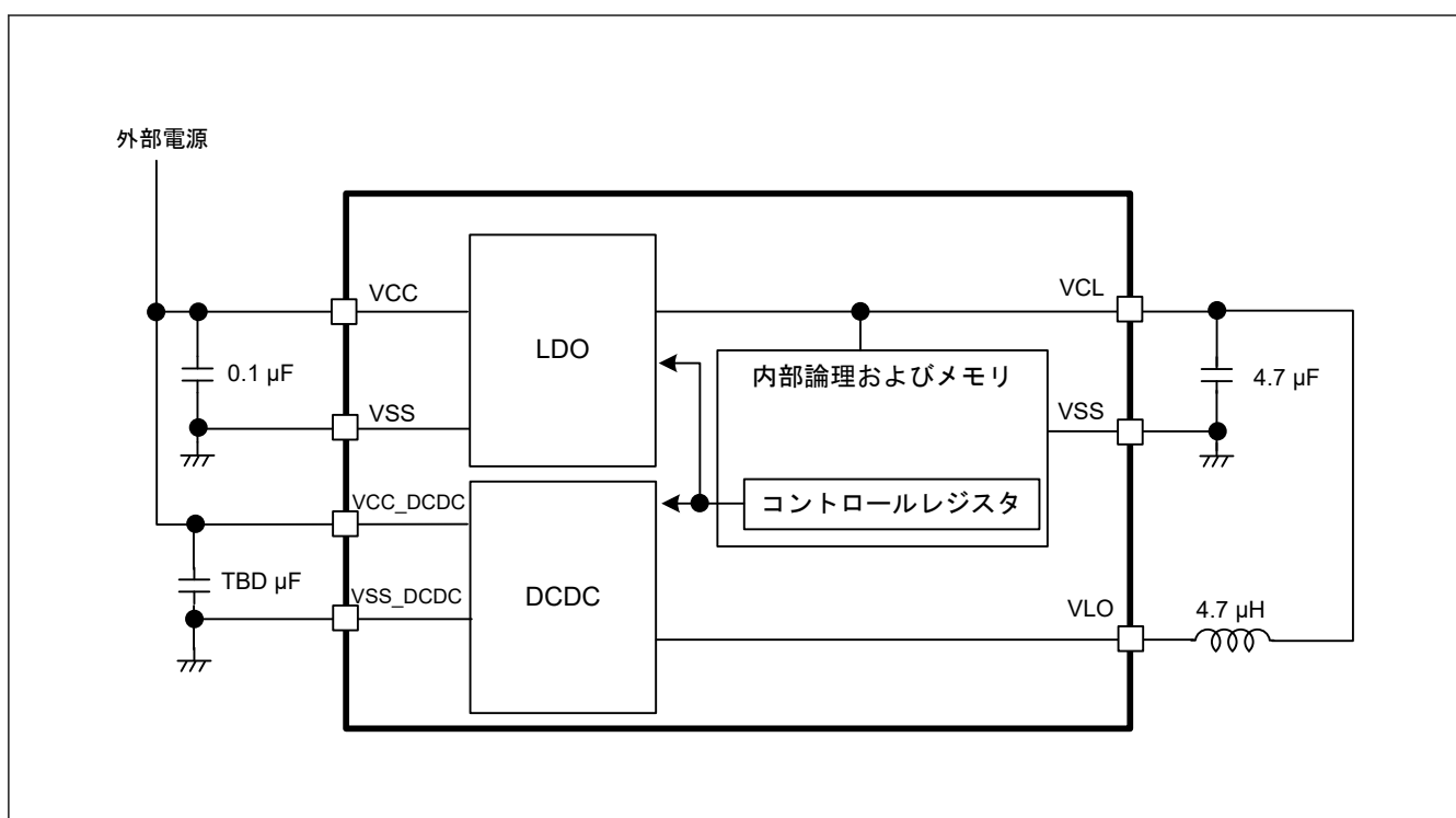
図 40.2 DCDC モード設定
