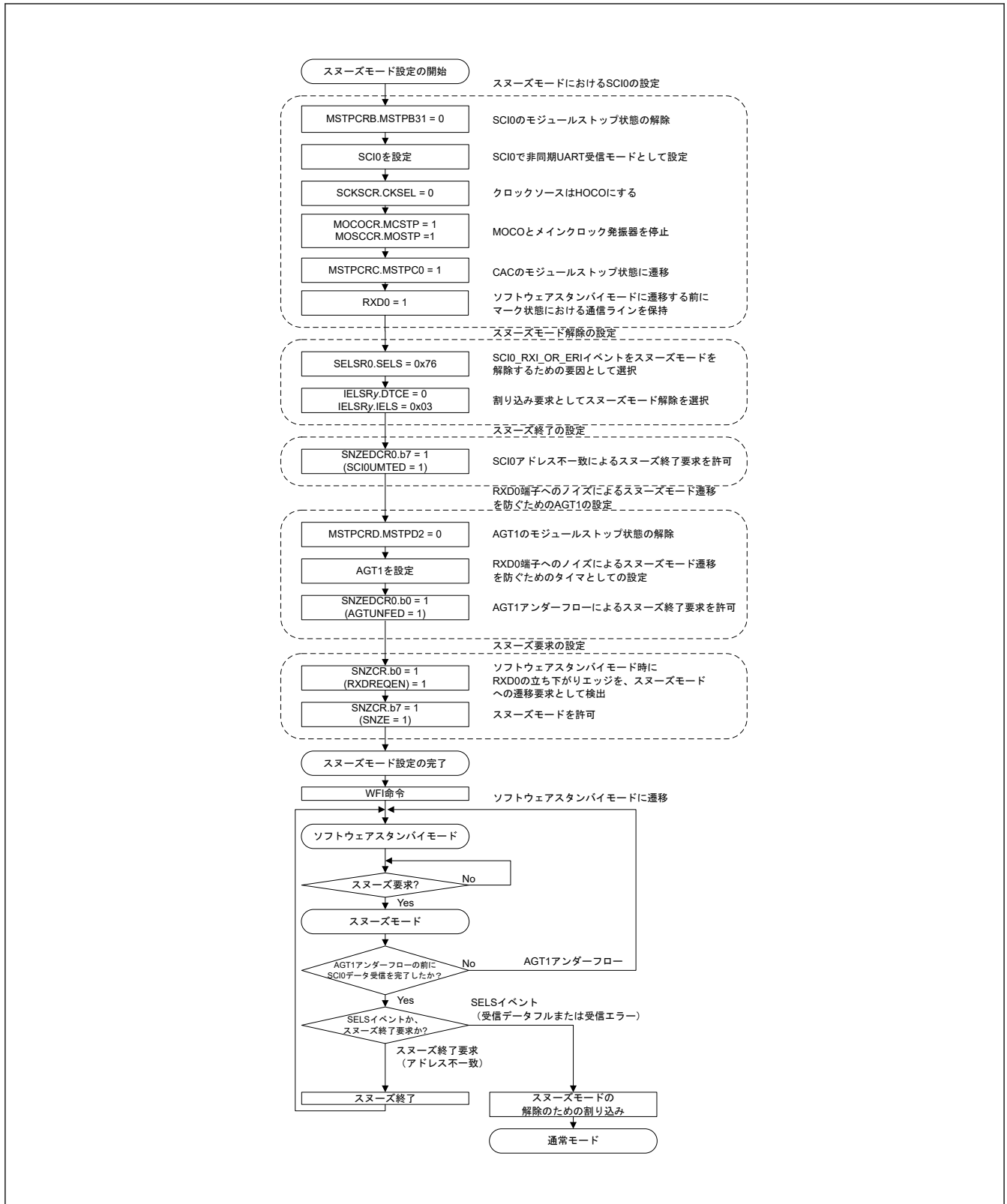
図 10.13 スヌーズモードエントリでSCI0を使用するための設定例
