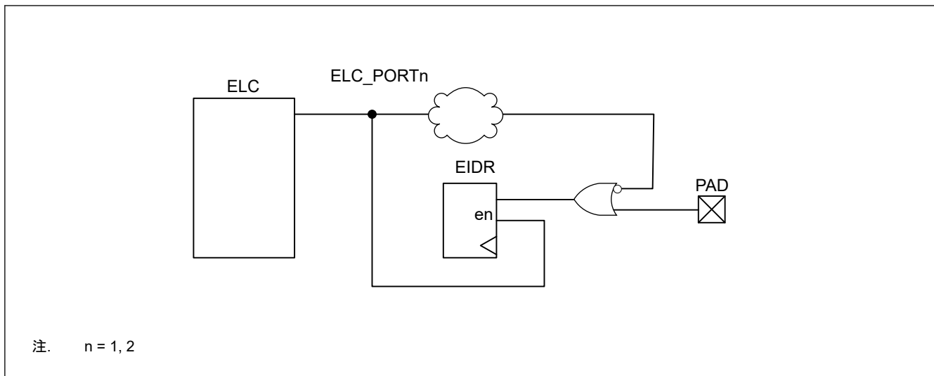
図 17.2 イベントポート入力データ
