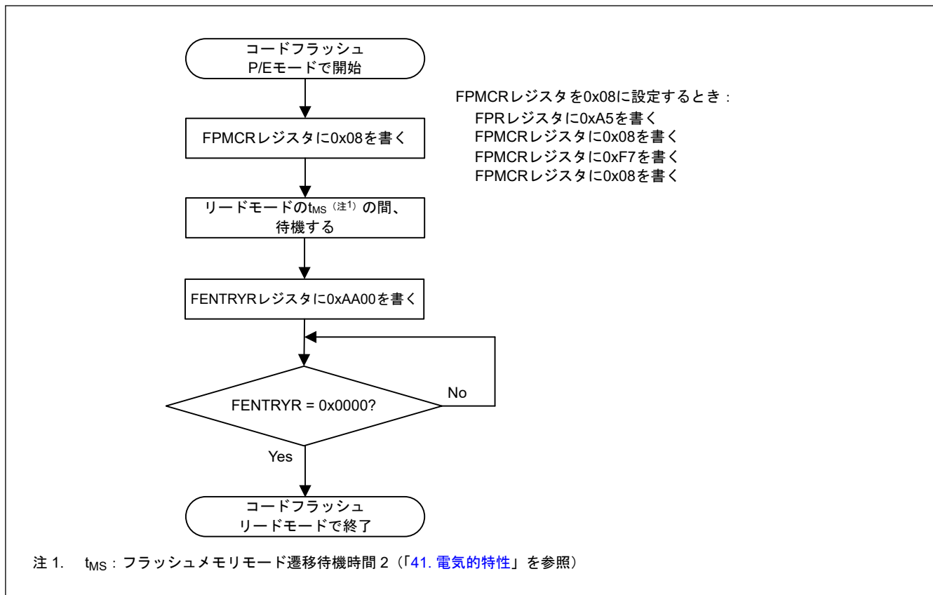
図 37.17 コードフラッシュ P/E モードから読み出しモードへの変更手順
