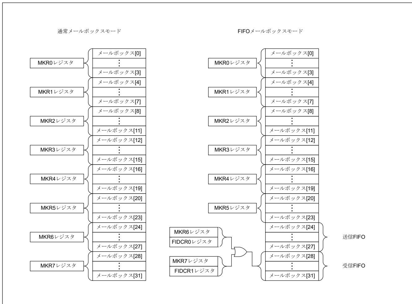
図 27.16 マスクレジスタとメールボックスの対応
