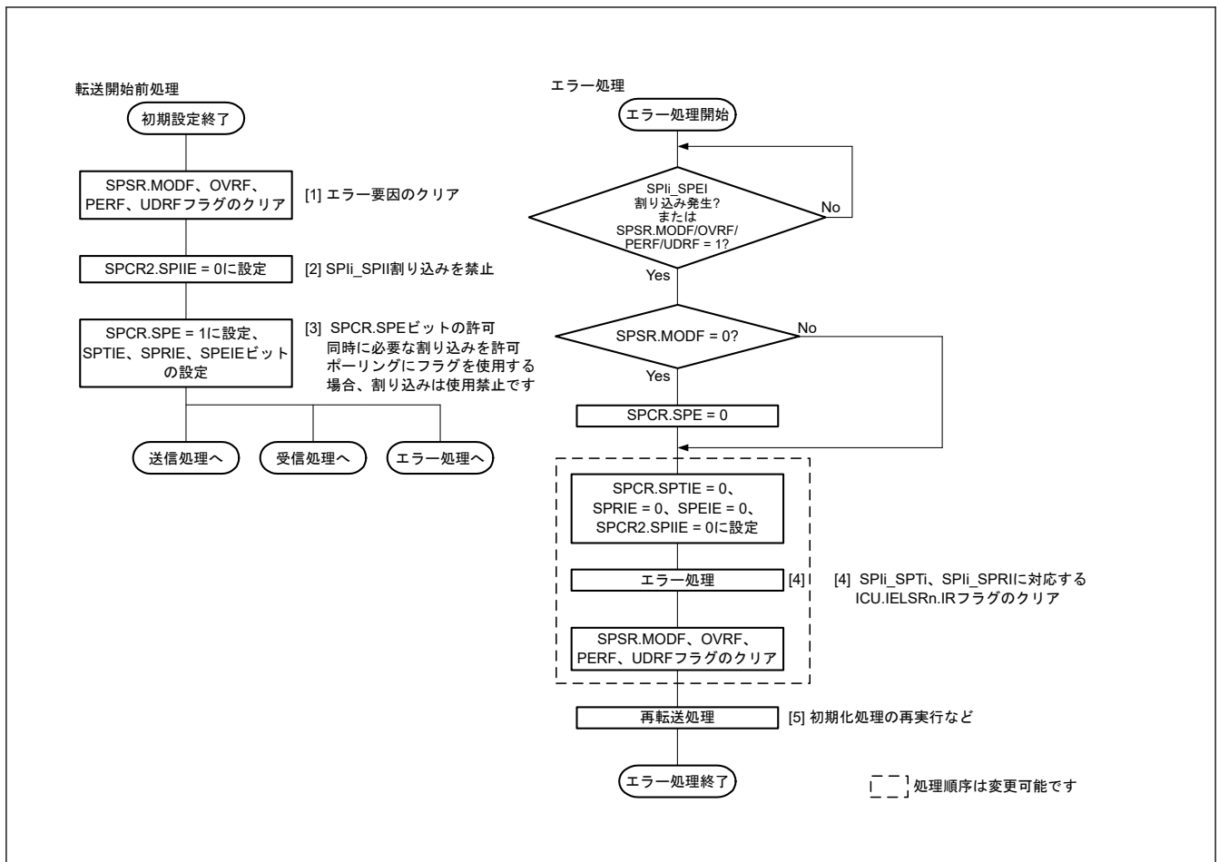
図 28.39 スレーブモードでのエラー処理フロー
