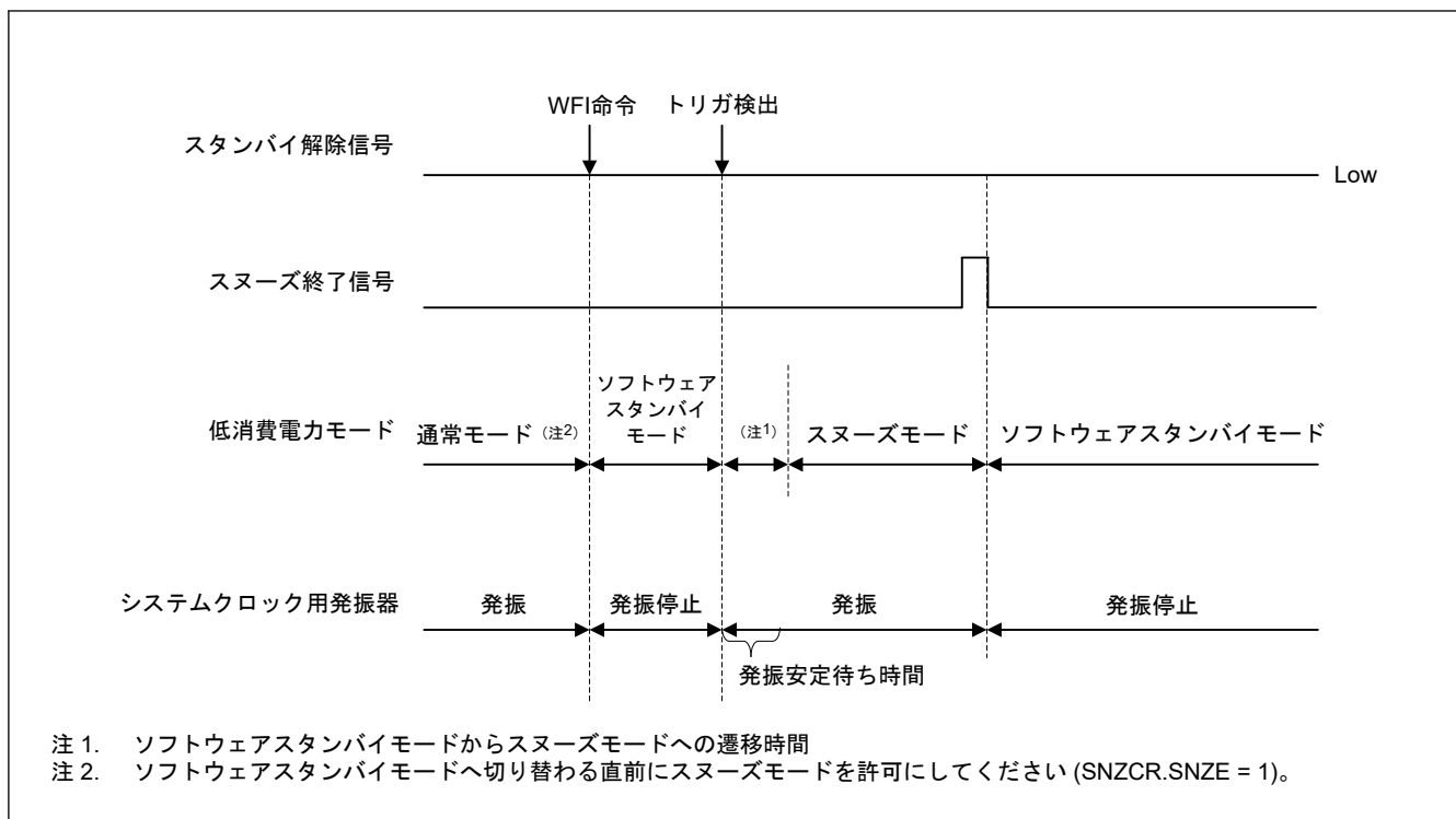
図 10.11 割り込み要求信号が発生しない場合のスリープモードの解除
