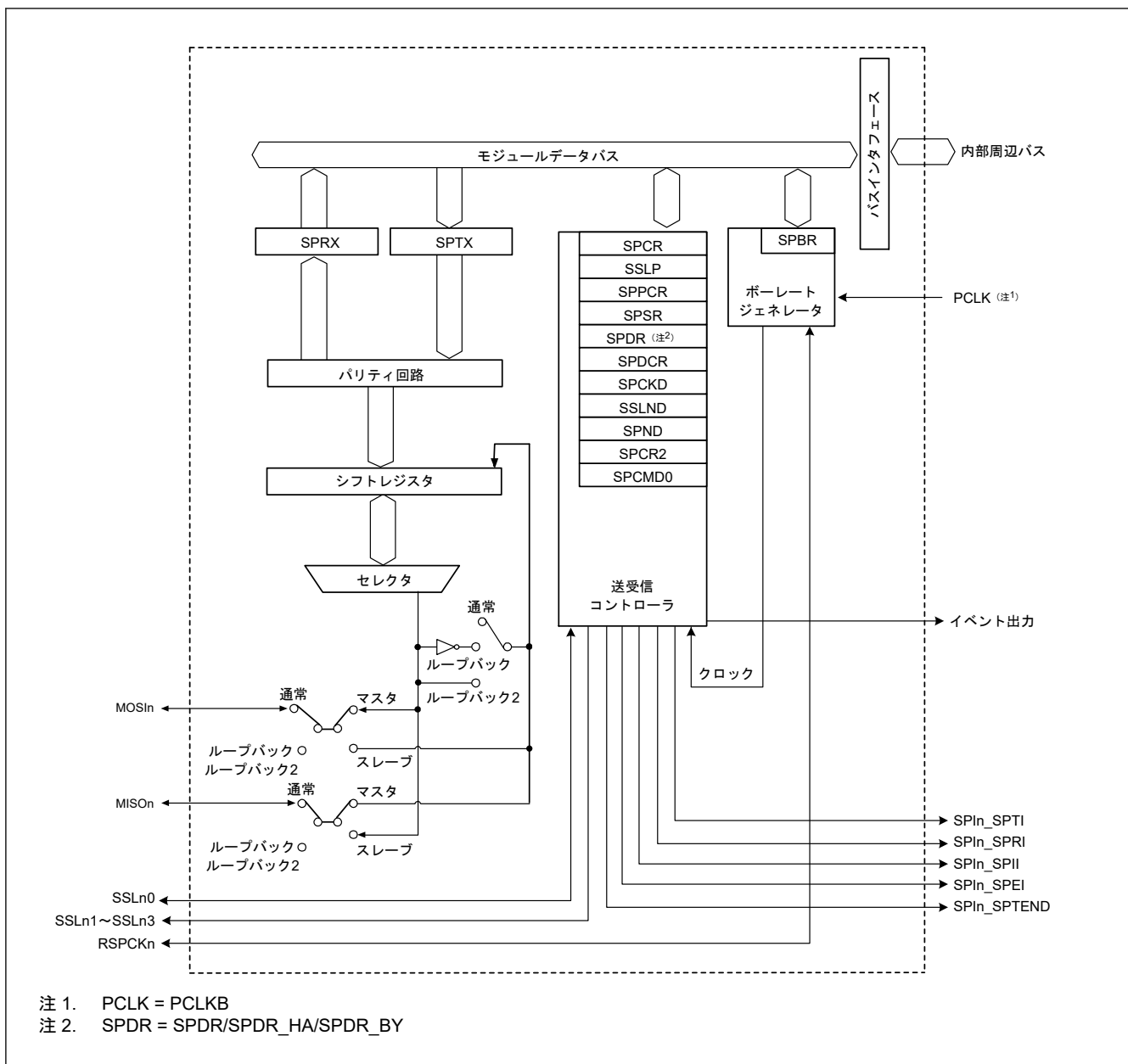
図 28.1 SPI のブロック図
