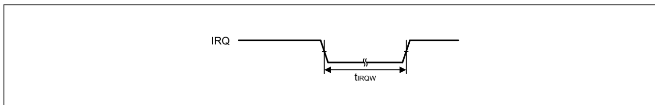
図 41.13 IRQ 割り込み入力タイミング
