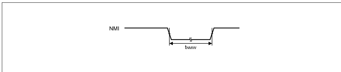
図 41.12 NMI 割り込み入力タイミング
