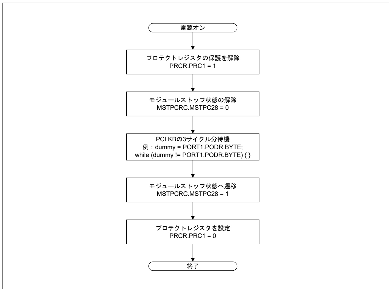
図 10.14 未使用回路の初期設定フロー例
