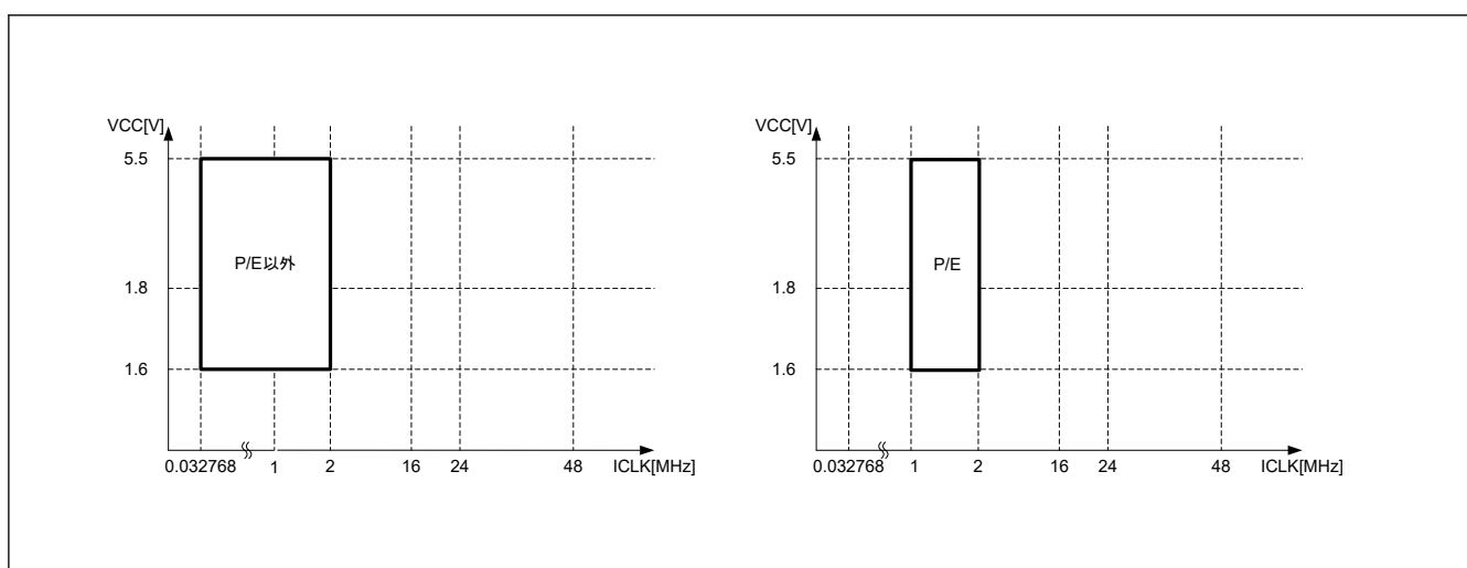
図 10.6 Low-speed モードにおける動作電圧と動作周波数
