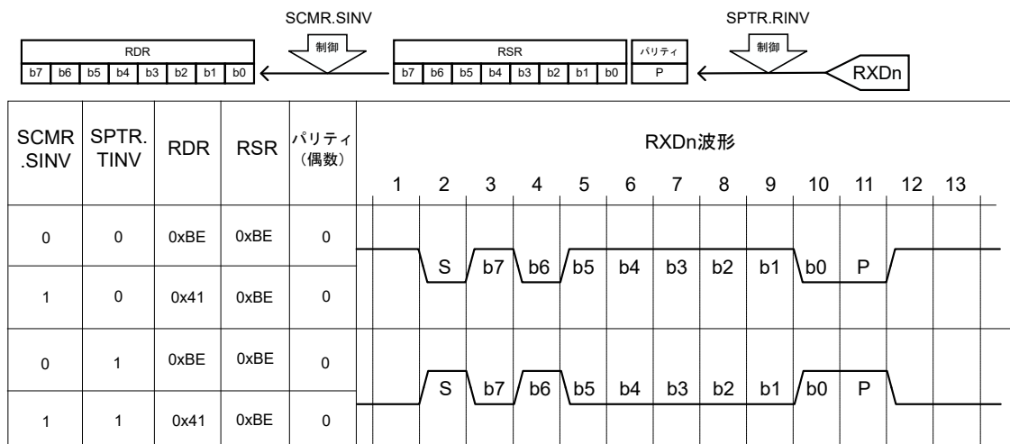
図 24.2 受信/送信データ制御の例
