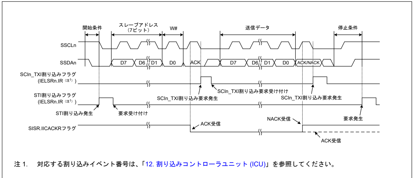
図 24.90 簡易 IIC モードにおけるマスタ送信の動作例 1 (7 ビットスレーブアドレス、送信割り込み、受信割り込み使用時)
