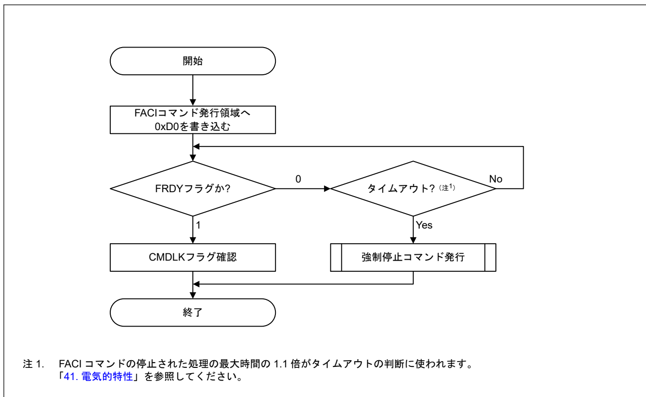
図 38.20 P/E レジュームコマンドの使用フロー
