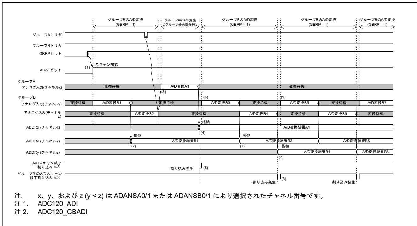
図 32.30 グループ優先動作例 1-5: グループ B のシングルスキャン連続動作 (ADGSPCR.GBRP = 1、ADGSPCR.LGRRS = 0 の場合)
