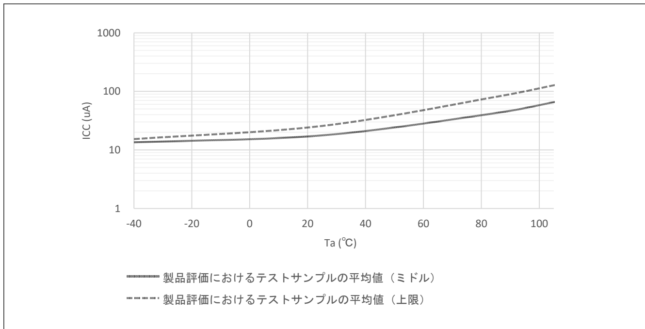
図 41.3 ディープソフトウェアスタンバイモード時の温度依存性、DPSBYCR.DEEPCUT[1:0] = 00b (参考データ)
