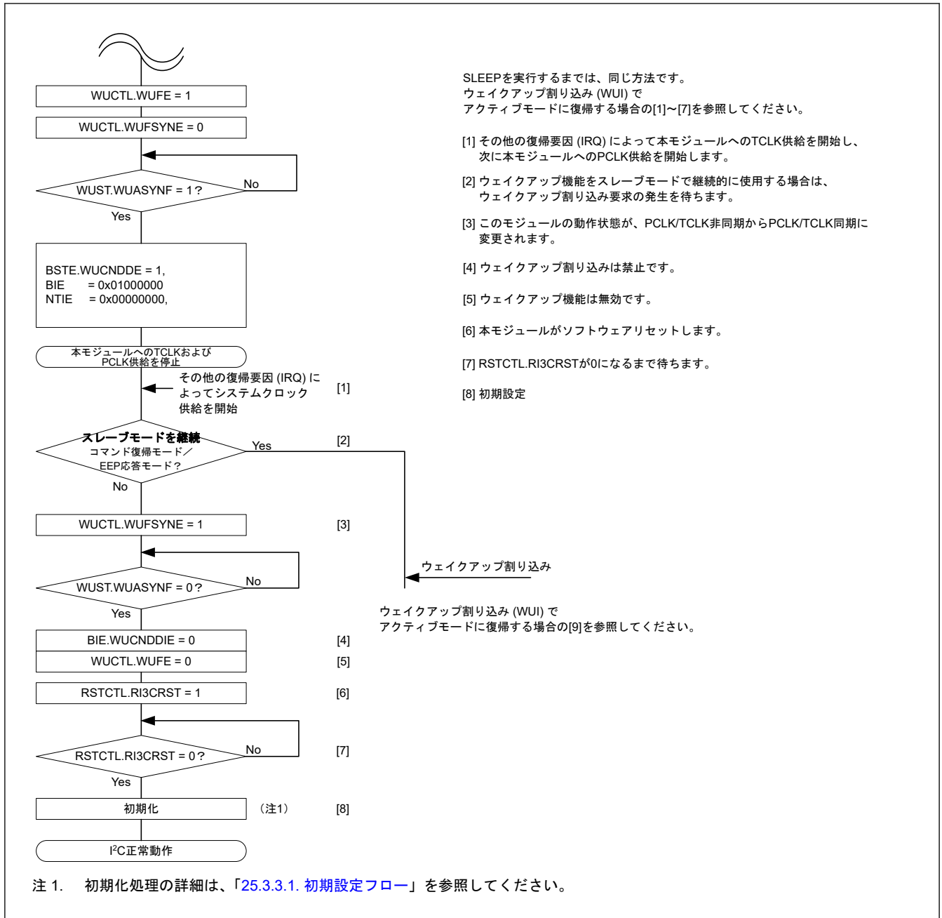
図 25.105 コマンドリカバリモードと EEP 応答モードの使用例 (他のリカバリ要因 (IRQ) によるウェイクアップリカバリの場合)
