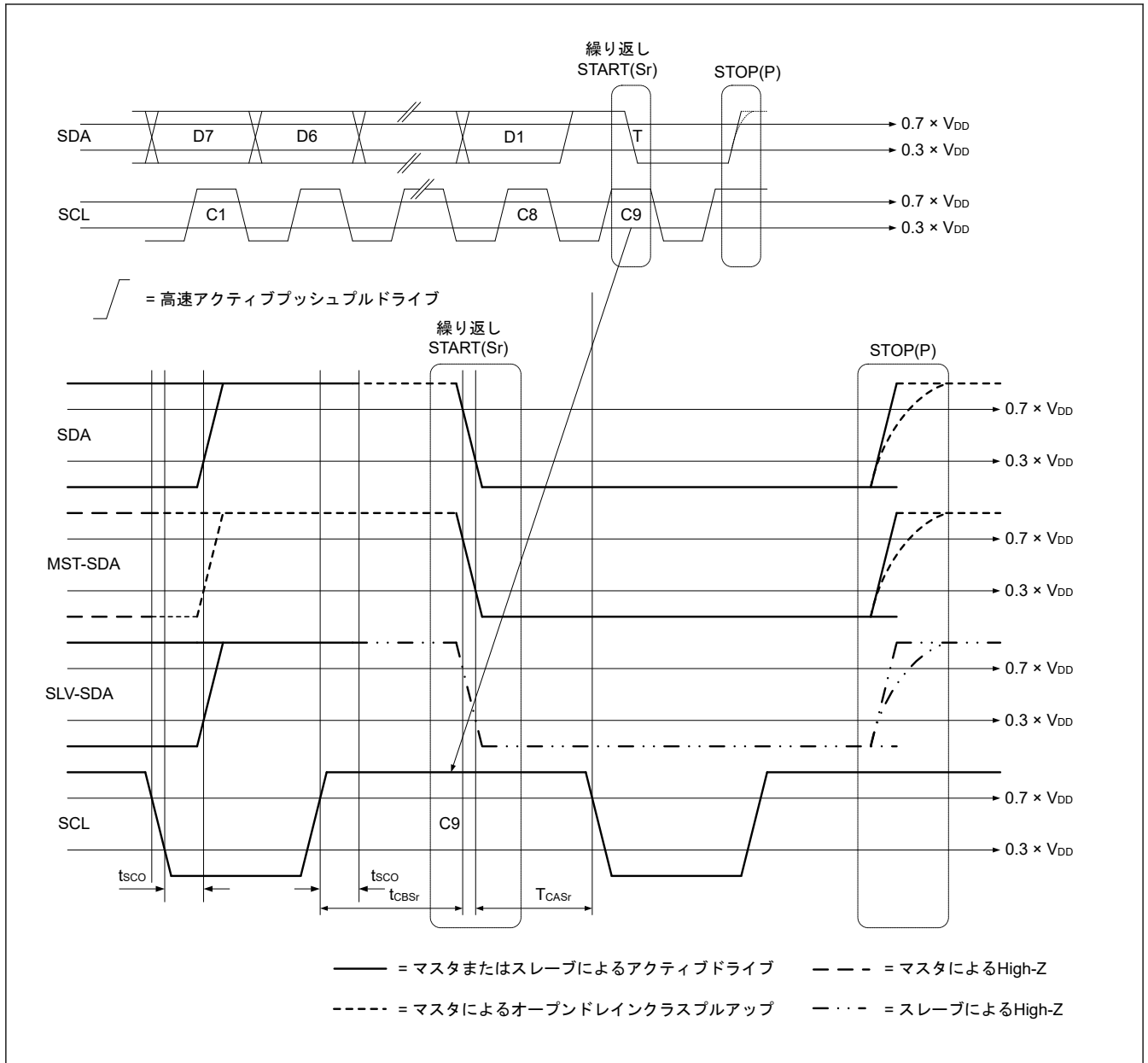
図 41.50 繰り返しのスタートコンディションおよびストップコンディションでのマスタ終了時のTビット読み出し
