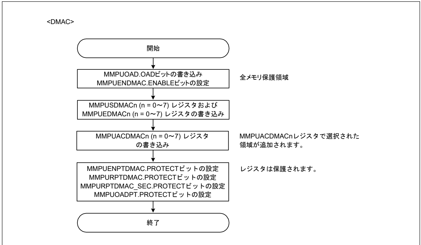
図 14.3 リセット後のバスマスタ MPU のレジスタ設定フロー
