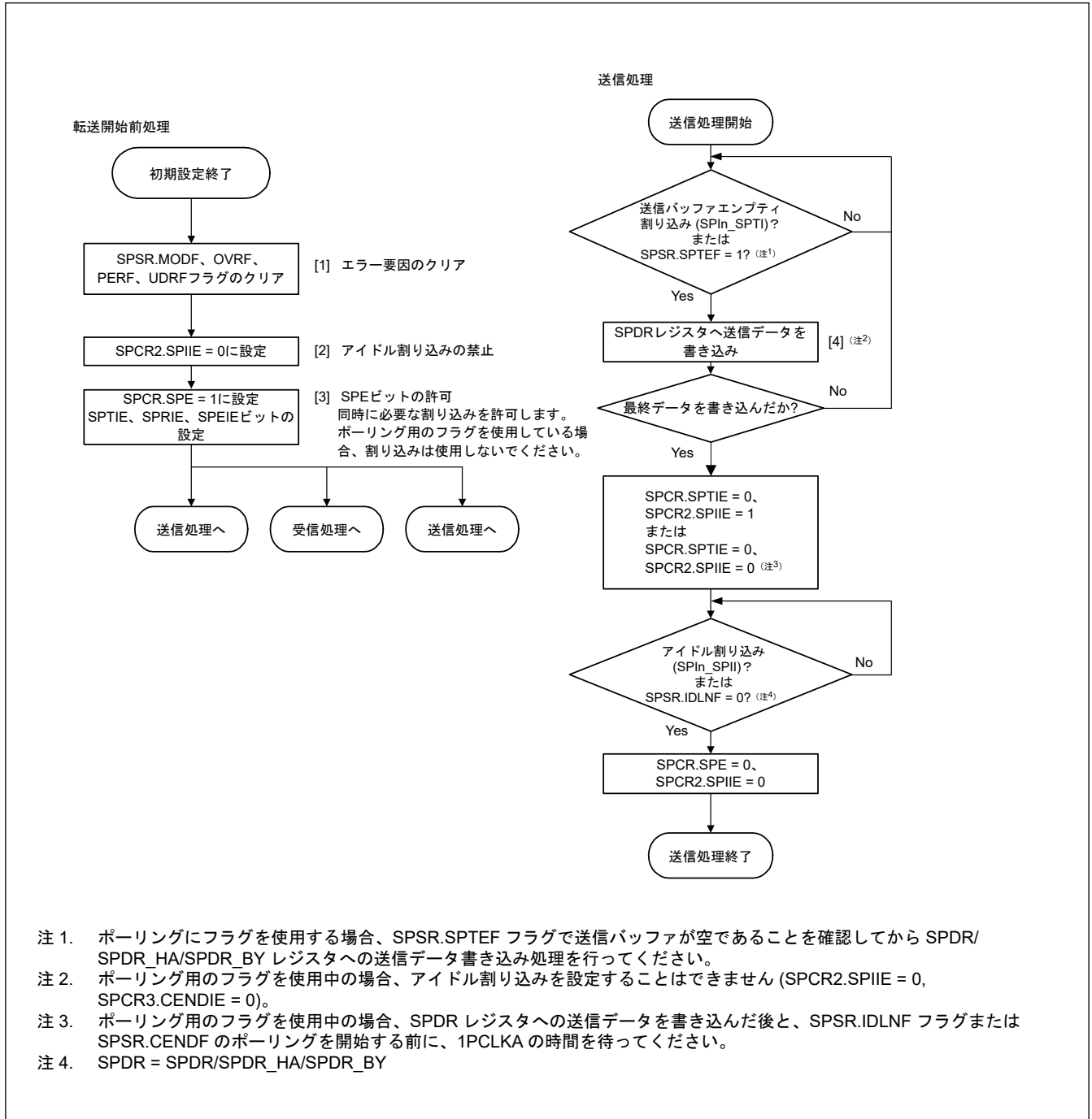
図 28.49 マスタモードでの送信フロー
