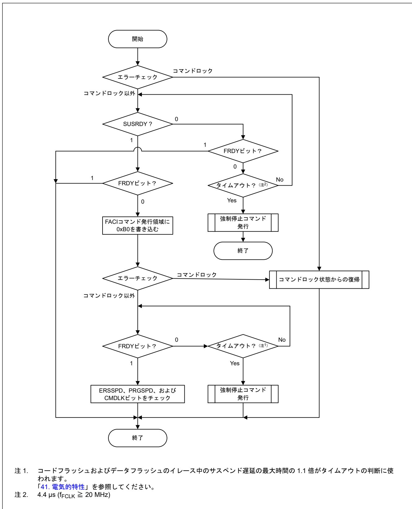
図 38.16 P/E サスペンドコマンドの使用フロー
