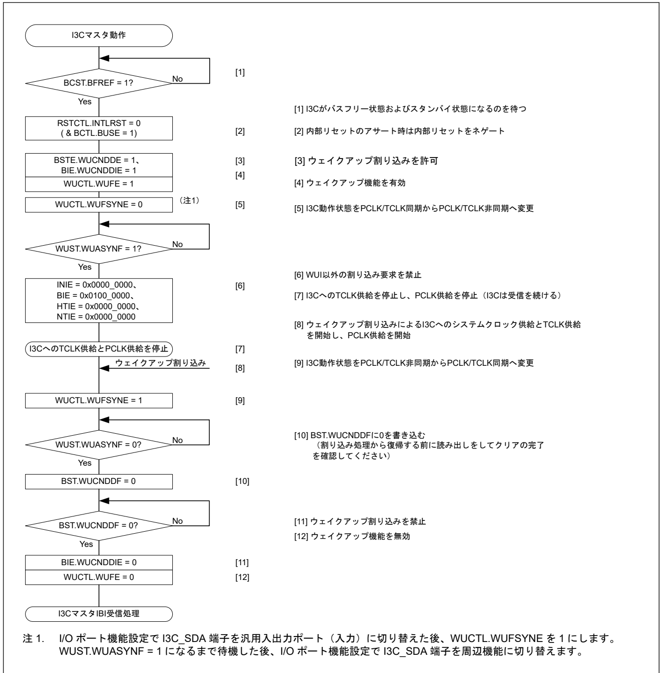
図 25.124 I3C マスタウェイクアップの使用例
