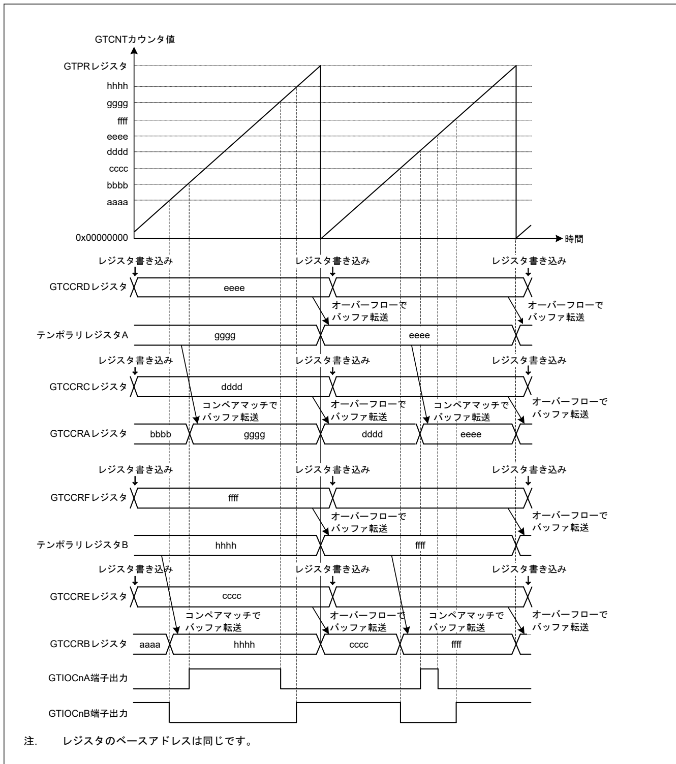
図 20.23 のこぎり波ワンショットパルスモードの動作例 (アップカウント、カウントスタート時に GTIOcNA 端子 = Low 出力 / GTIOcNB 端子 = High 出力、GTCCRr/GTCCRb レジスタのコンペアマッチ時に トグル出力、周期の終わりで出力保持の場合)
