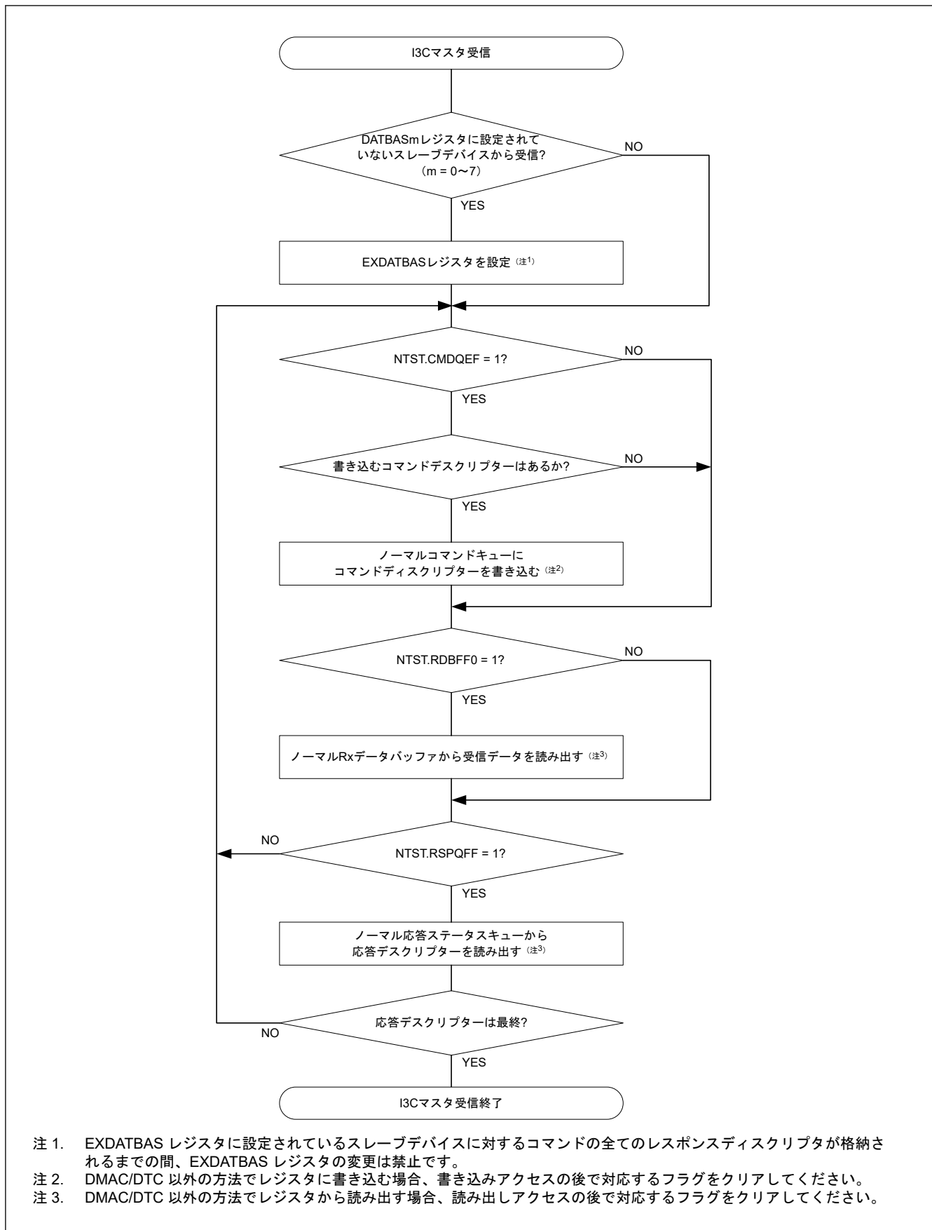
図 25.120 I3C マスタ受信のフローチャート例 (通常 FIFO バッファ転送)
