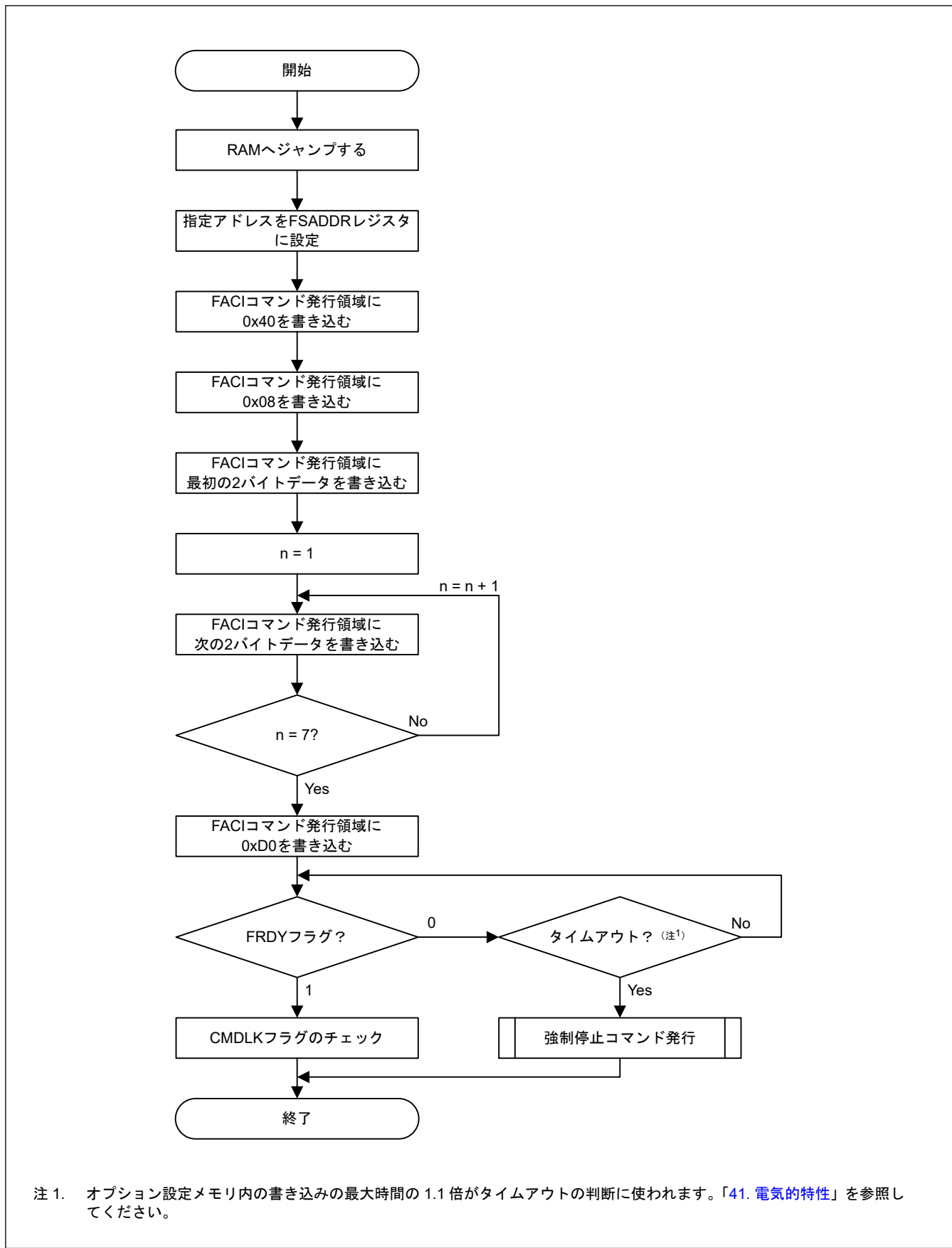
図 38.24 コンフィグレーション設定コマンドの使用フロー
