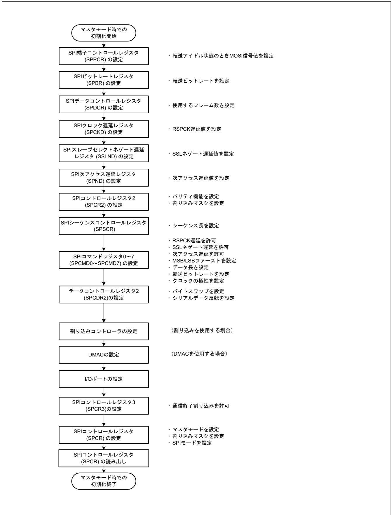
図 28.59 マスタモード時のクロック同期式動作の初期化フロー例
