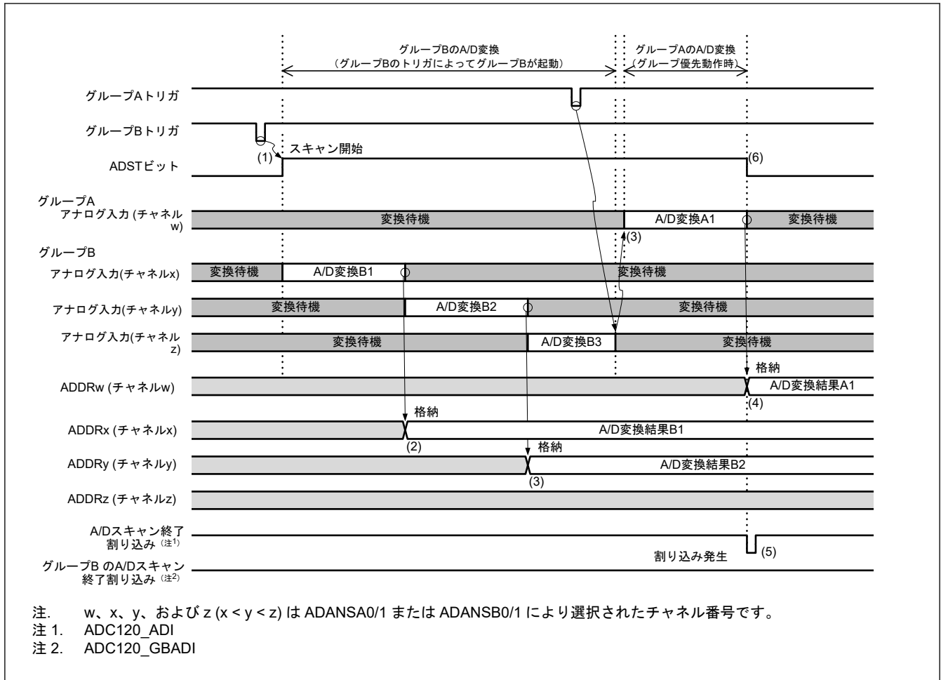
図 32.29 グループ優先動作例 1-4：グループ B スキャン中のグループ A トリガ入力、再スキャンなし (ADGSPCR.GBRSCN = 0、ADGSPCR.GBRP = 0、および ADGSPCR.LGRRS = 0 の場合)
