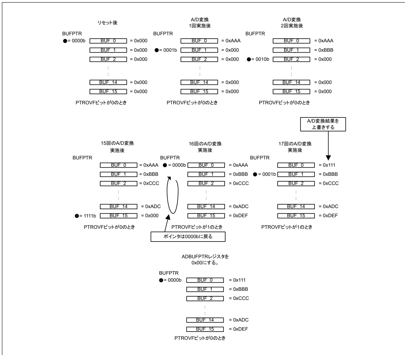
図 32.40 データバッファ、ポインタ、およびオーバーフローフラグの動作概略図
