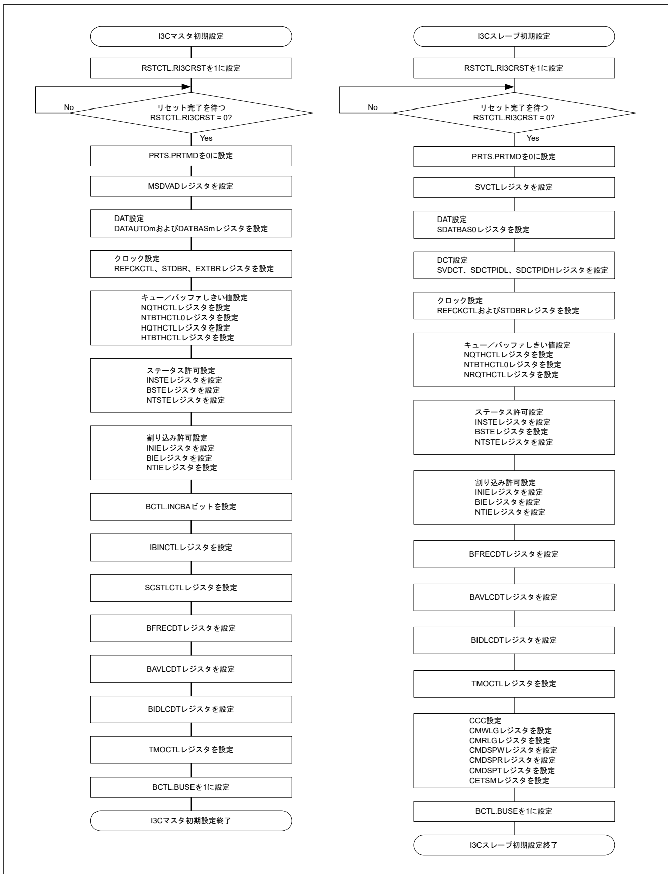
図 25.114 I3C の初期化フローチャート例
