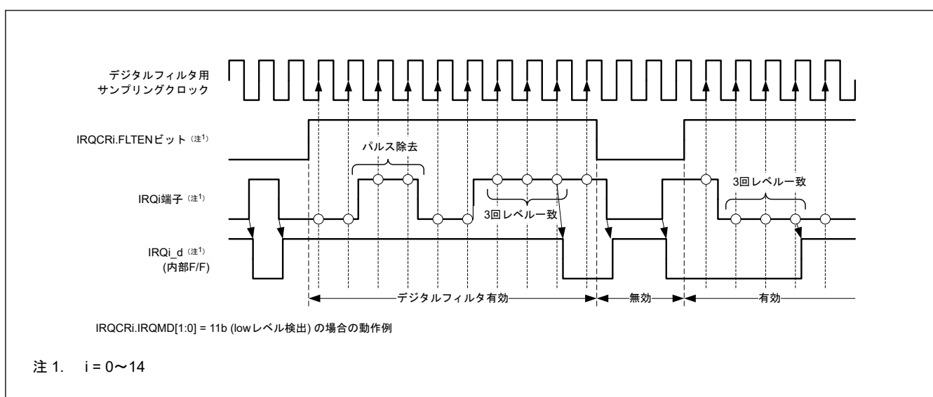
図 12.4 デジタルフィルタの動作例
