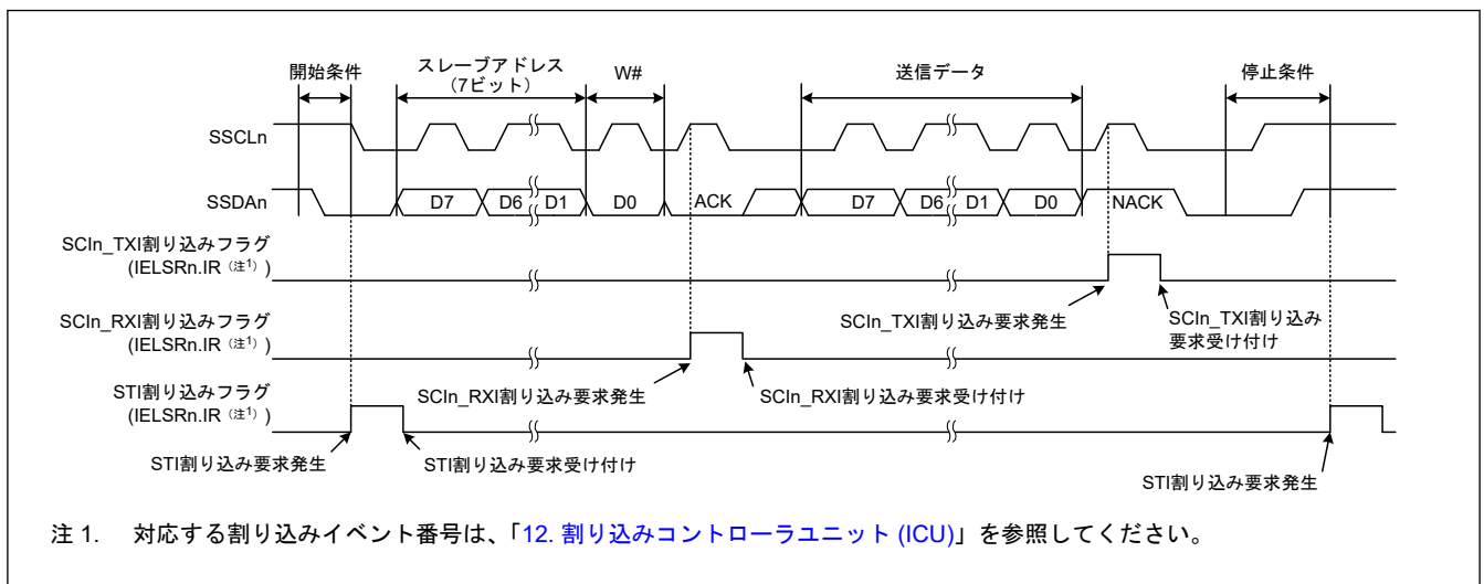
図 24.91 簡易 IIC モードにおけるマスタ送信の動作例 2 (7 ビットスレーブアドレス、ACK 割り込み、NACK 割り込み使用時)
