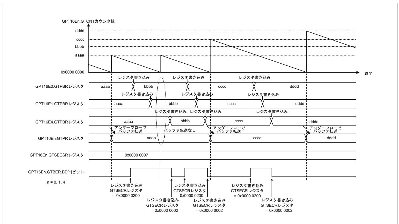
図 20.80 バッファ動作禁止の複数チャンネルの動作例 (のこぎり波、シングルバッファ動作)
