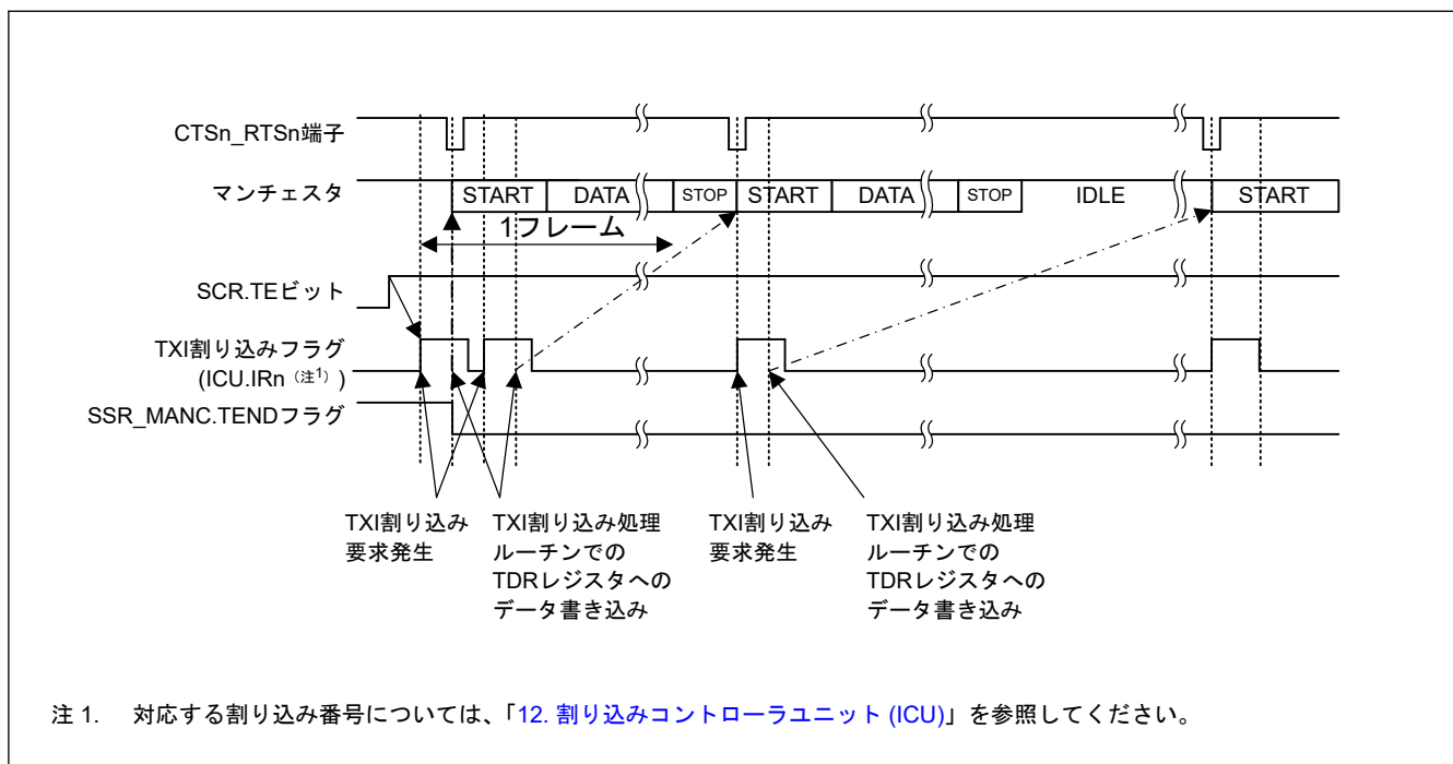
図 24.54 マンチェスタモードにおけるシリアル送信の送信開始動作の例 (プレフィスなし、CTS 機能あり)
