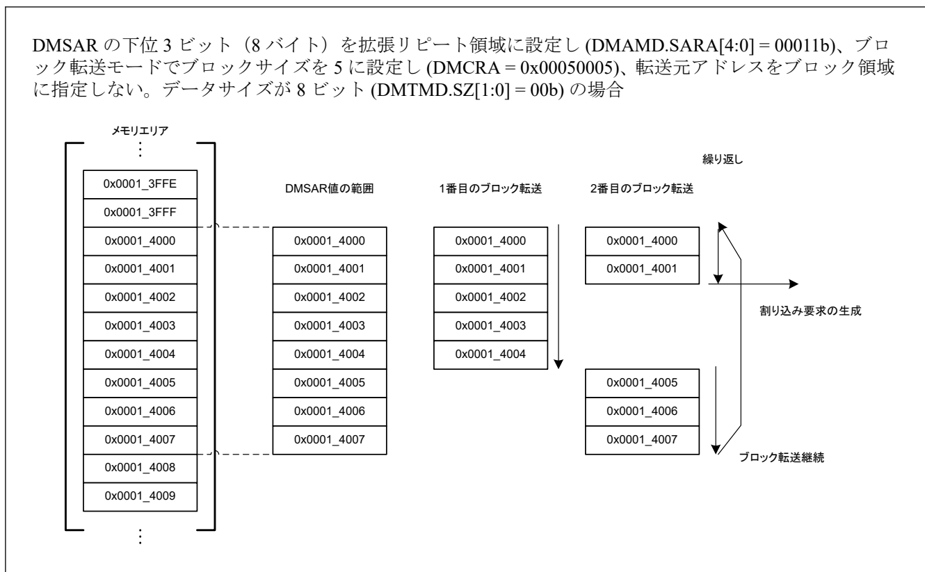
図 15.8 ブロック転送モードにおける拡張リピート領域機能の使用例
