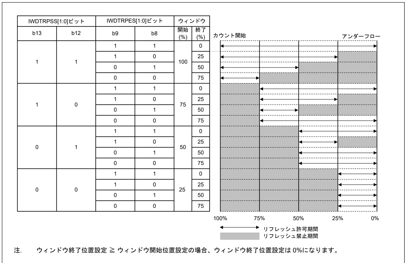
図 23.2 IWDRPSS[1:0]および IWDTRPES[1:0]ビットとリフレッシュ許可期間
