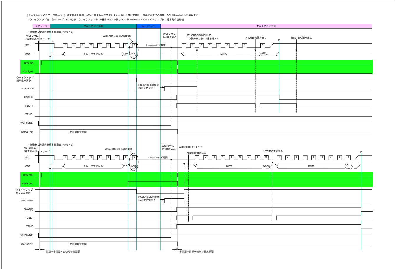
図 25.101 ノーマル WU モード 1 のタイミング
