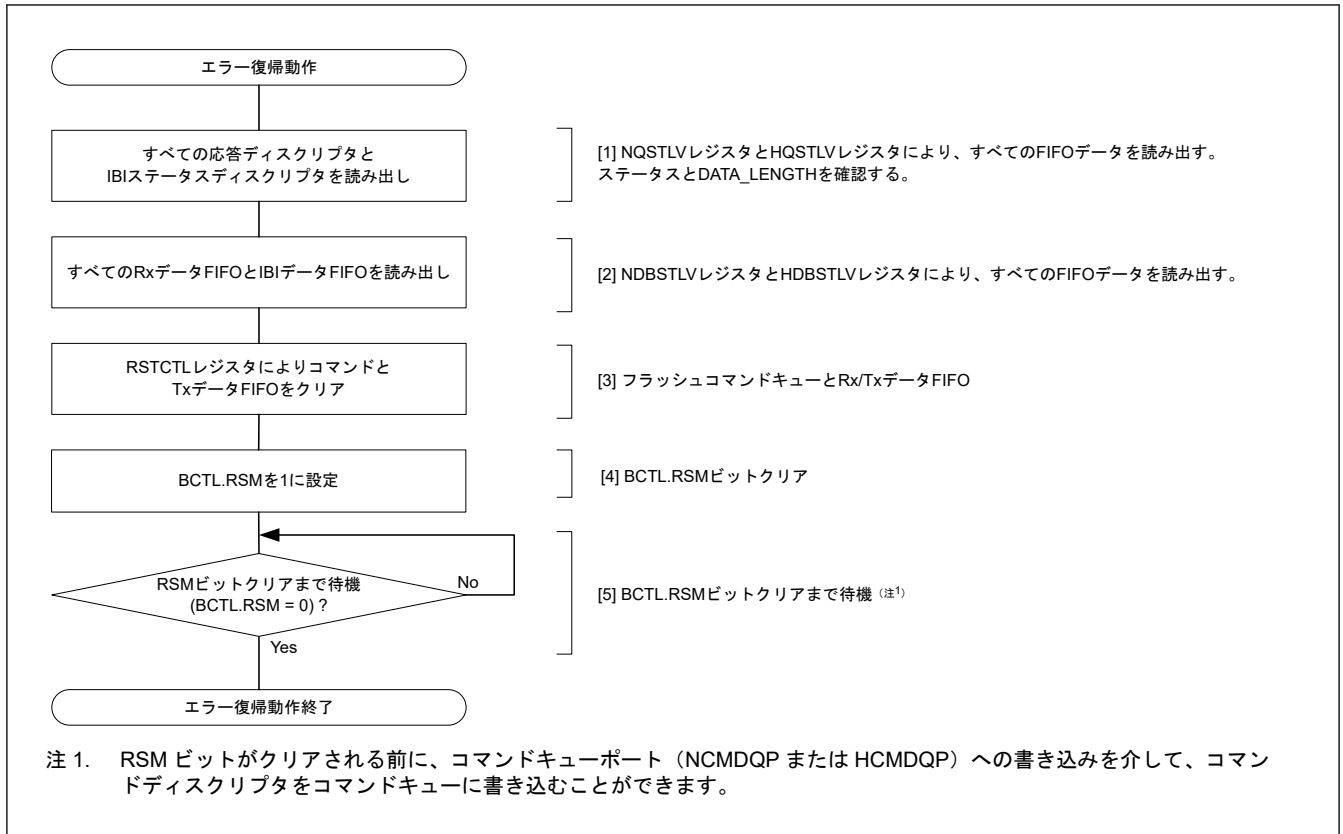
図 25.95 I3C マスタのエラー復帰動作フローの例
