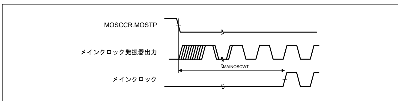
図 41.8 メインクロック発振開始タイミング
