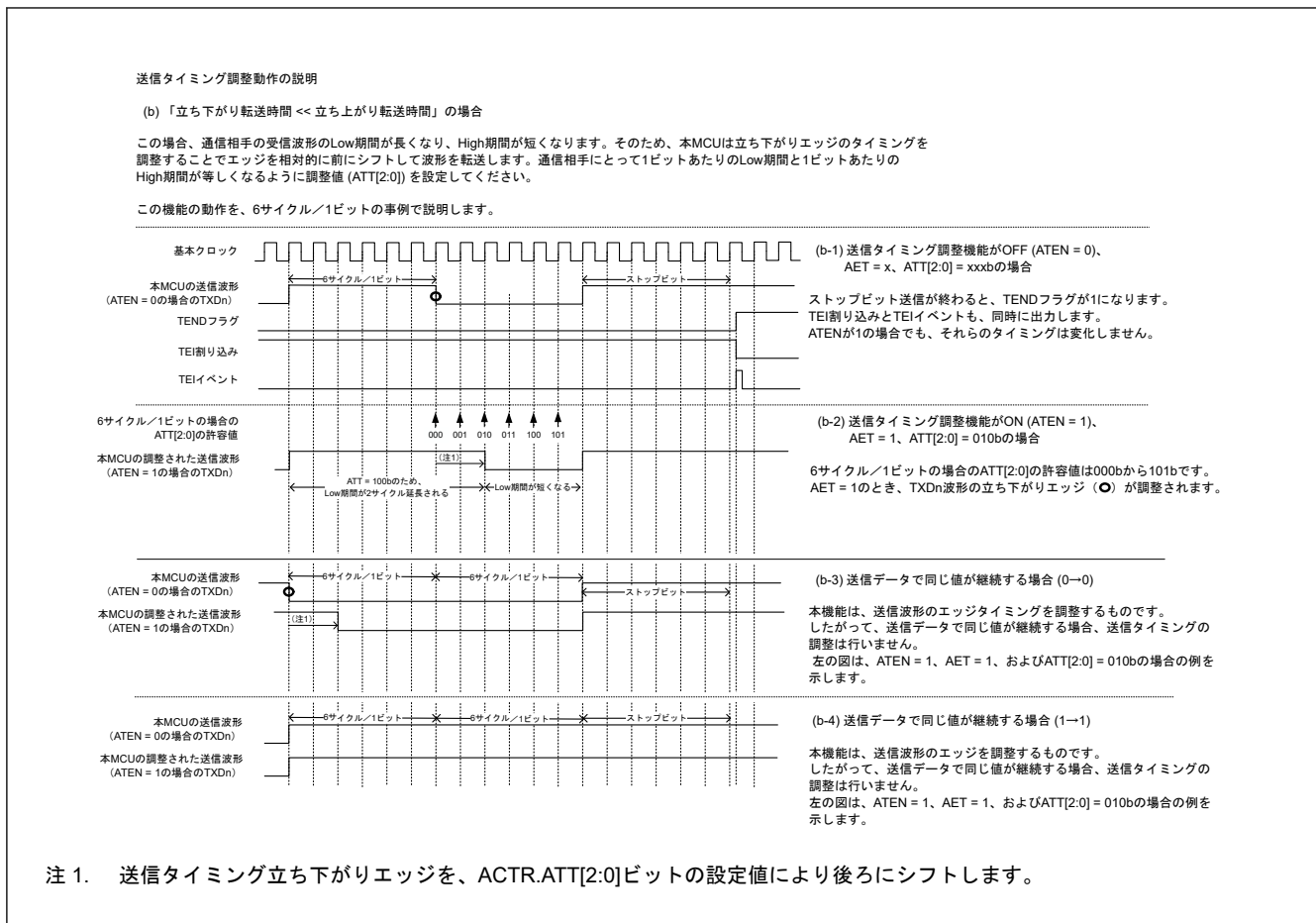
図 24.36 AET が 1 の場合の送信タイミング調節動作の説明
