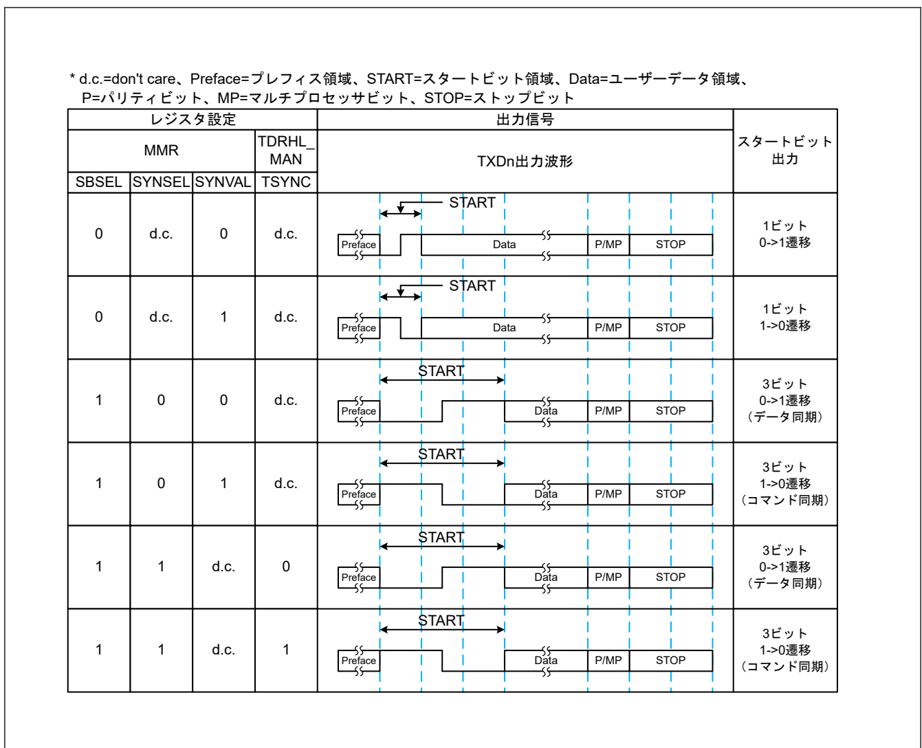
図 24.49 送信時のスタートビット領域に関する設定とフォーマット
