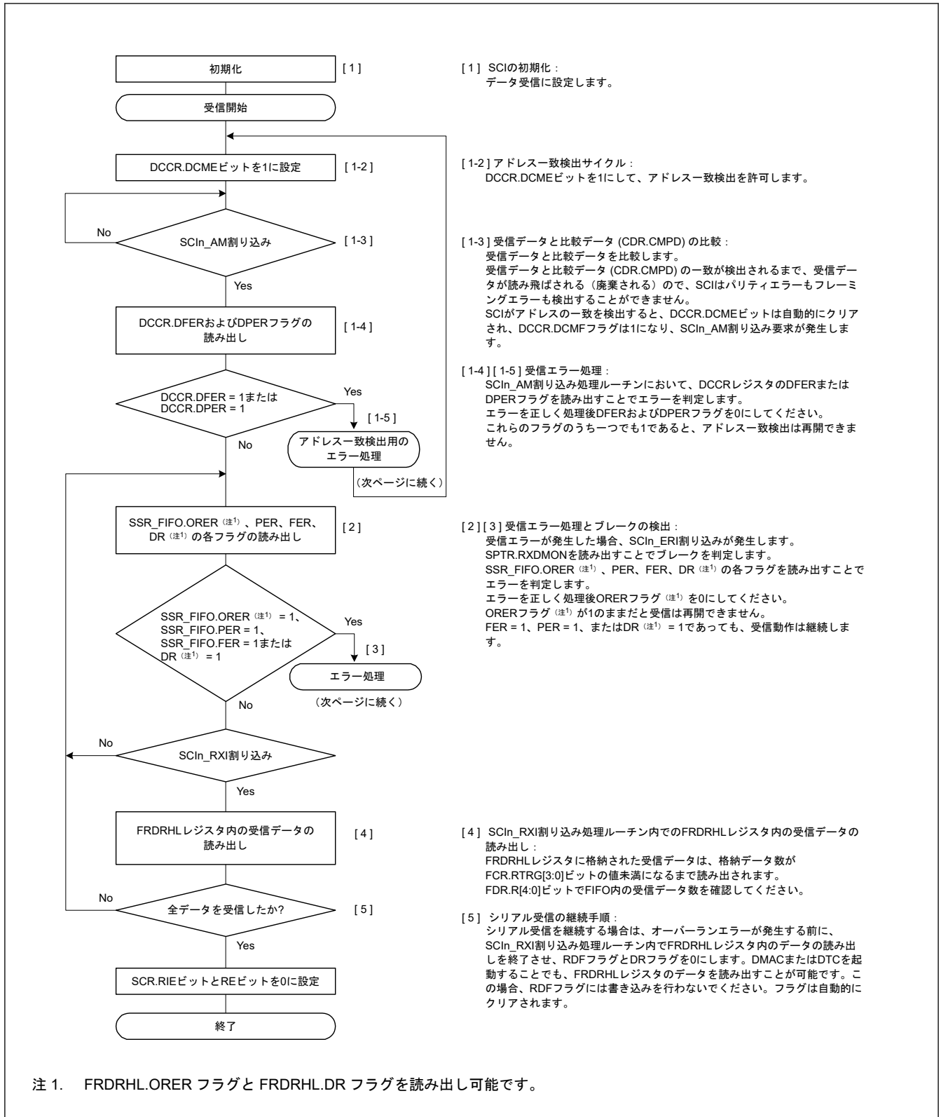
図 24.25 調歩同期式モードにおけるシリアル受信のフローチャート例 (FIFO 選択、アドレス一致検出有効時) (1)
