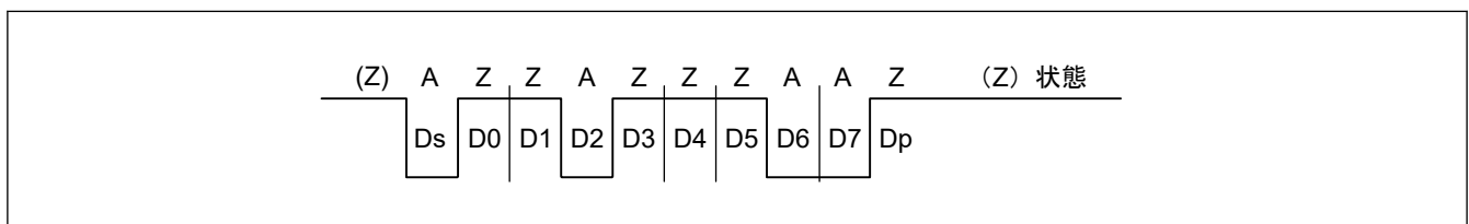
図 24.76 ダイレクトコンベンション (SCMR.SDIR ビット = 0、SCMR.SINV ビット = 0、SMR_SMCI.PM ビット = 0)
