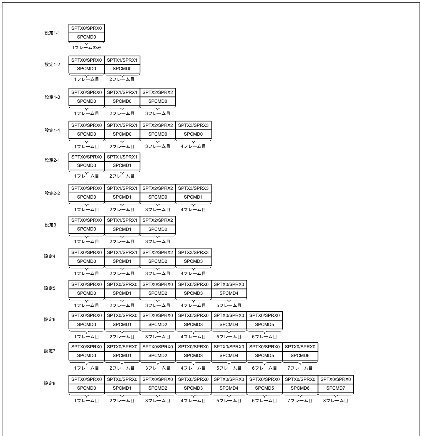
図 28.58 シーケンス動作時の SPI コマンドレジスタと送受信バッファの対応関係
