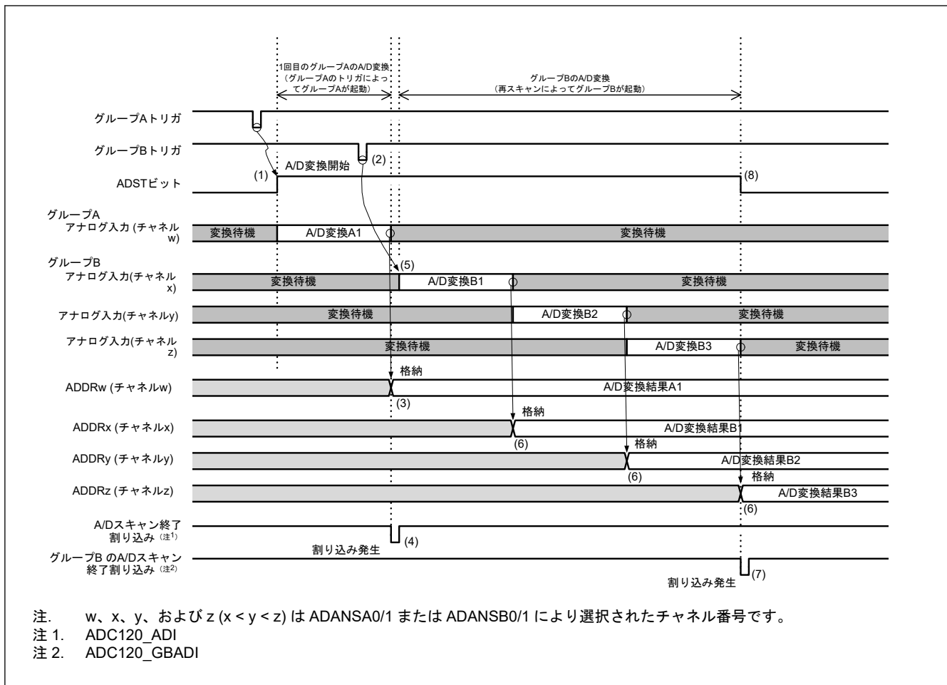
図 32.28 グループ優先動作例 1-3：グループ A スキャン中のグループ B トリガ入力、再スキャンあり (ADGSPCR.GBRSCN = 1、ADGSPCR.GBRP = 0、および ADGSPCR.LGRRS = 0 の場合)
