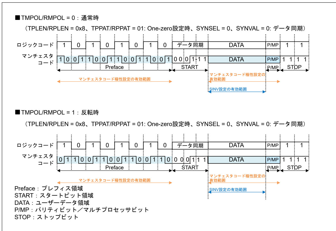
図 24.61 マンチェスタコード極性設定の有効範囲
