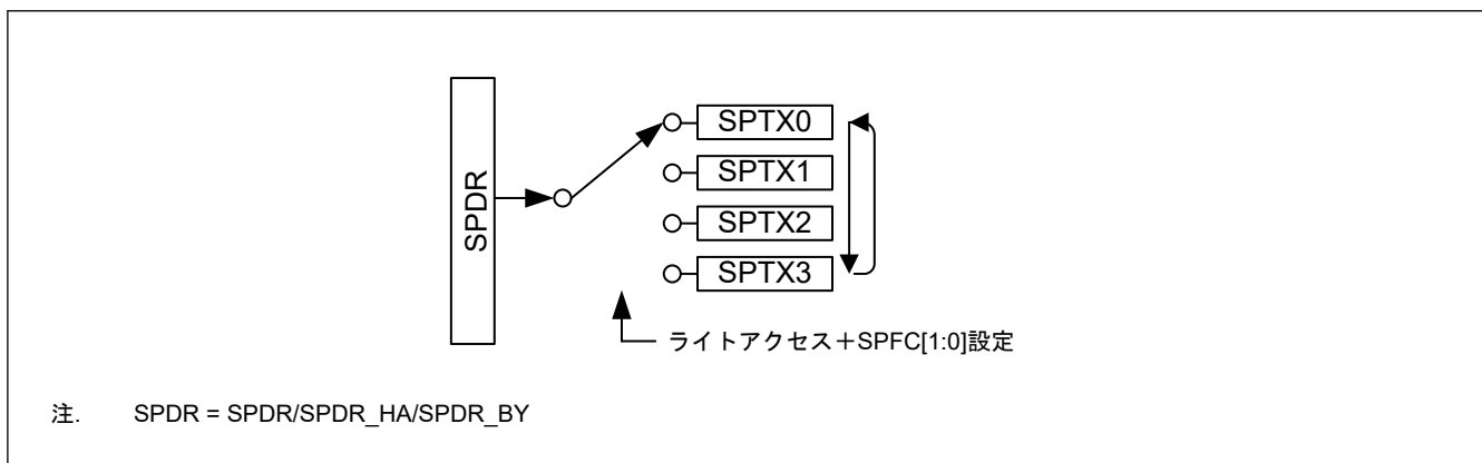
図 28.3 書き込み時の SPDR/SPDR_HA/SPDR_BY レジスタの構成図
