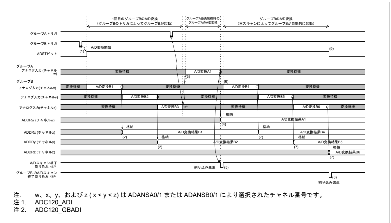
図 32.26 グループ優先動作例 1-1：グループ B スキャン中のグループ A トリガ入力、再スキャンあり (ADGSPCR.GBRSCN = 1、ADGSPCR.GBRP = 0、および ADGSPCR.LGRRS = 0 の場合)
