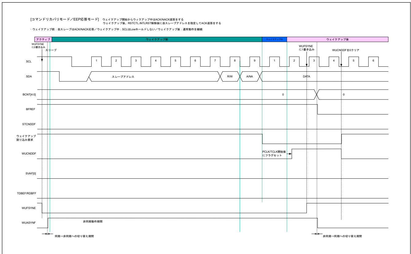
図 25.106 コマンドリカバリモードとEEP応答モードのタイミング
