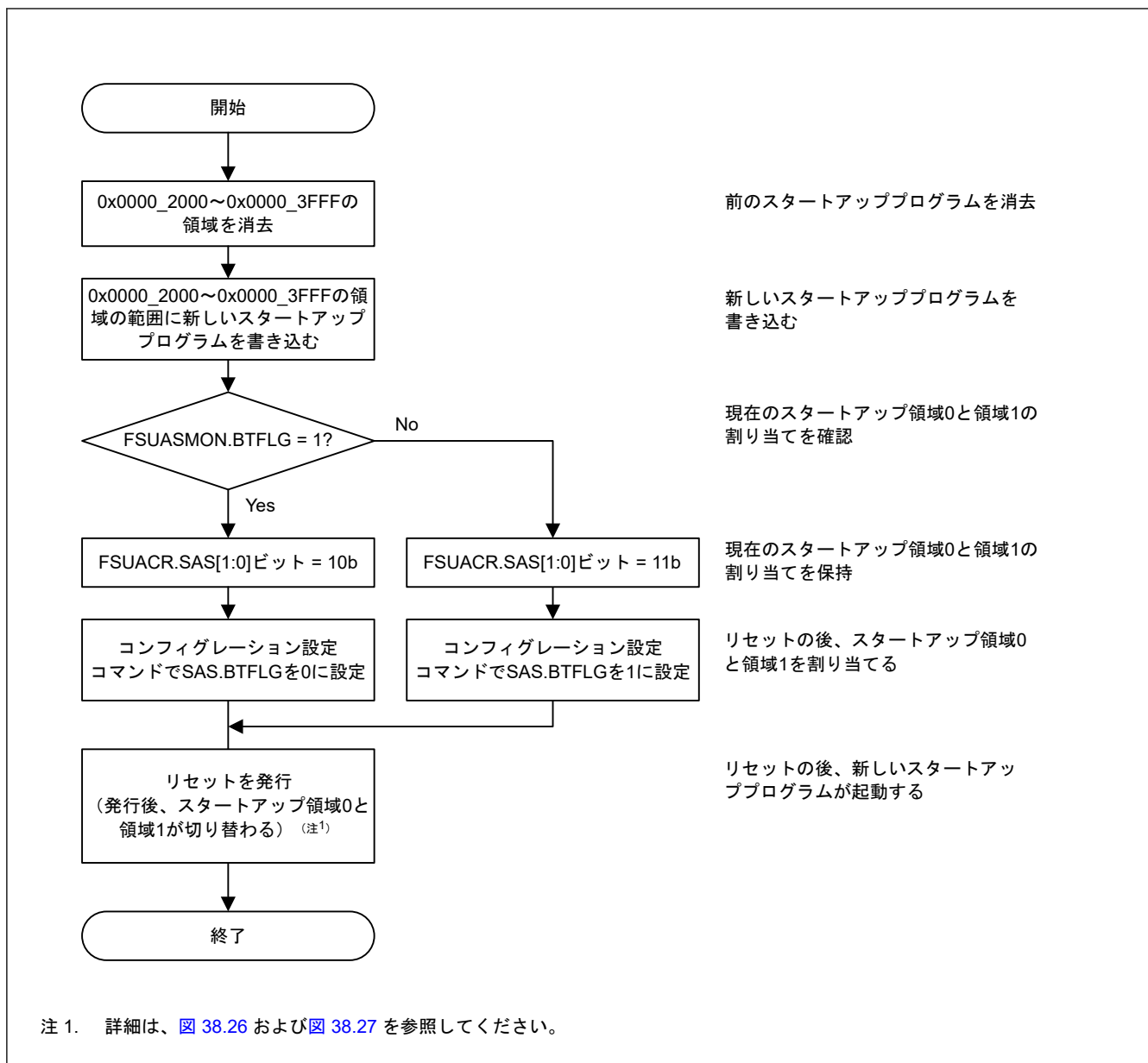
図 38.28 スタートアッププログラムプロテクションの概念
