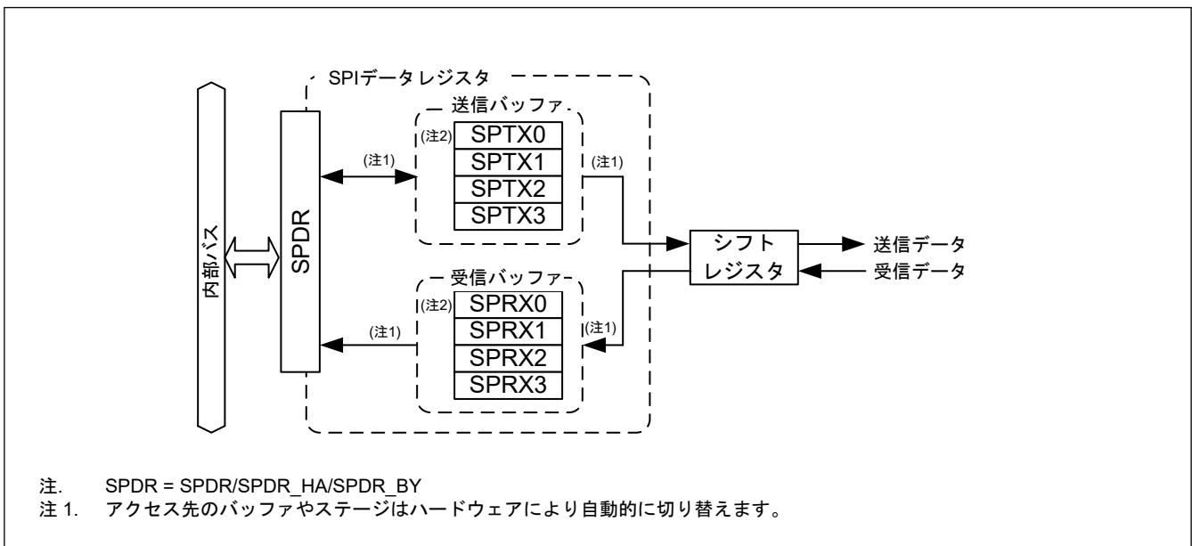
図 28.2 SPDR/SPDR_HA/SPDR_BY レジスタの構成図
