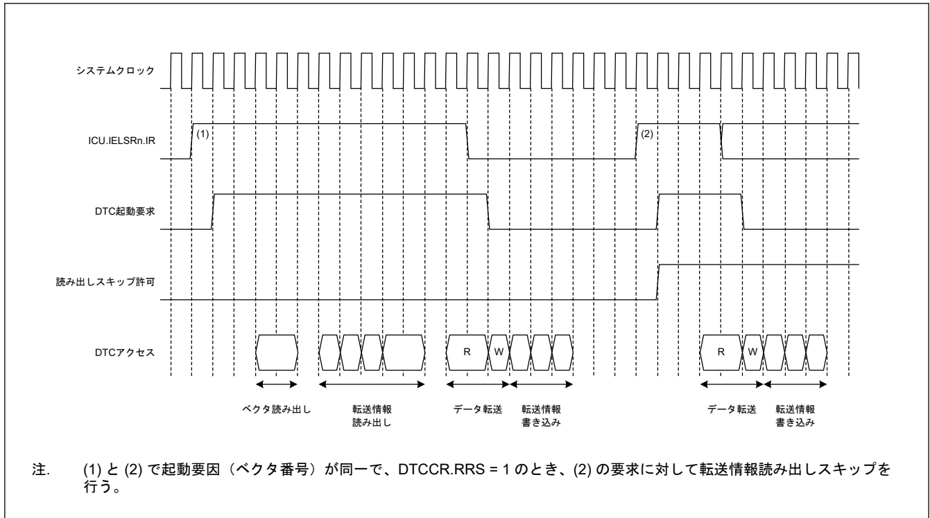
図 16.12 転送情報リードスキップ実行時の動作例(ベクタ、転送情報、転送先データがSRAMにあり、転送元データが周辺モジュールにある場合)
