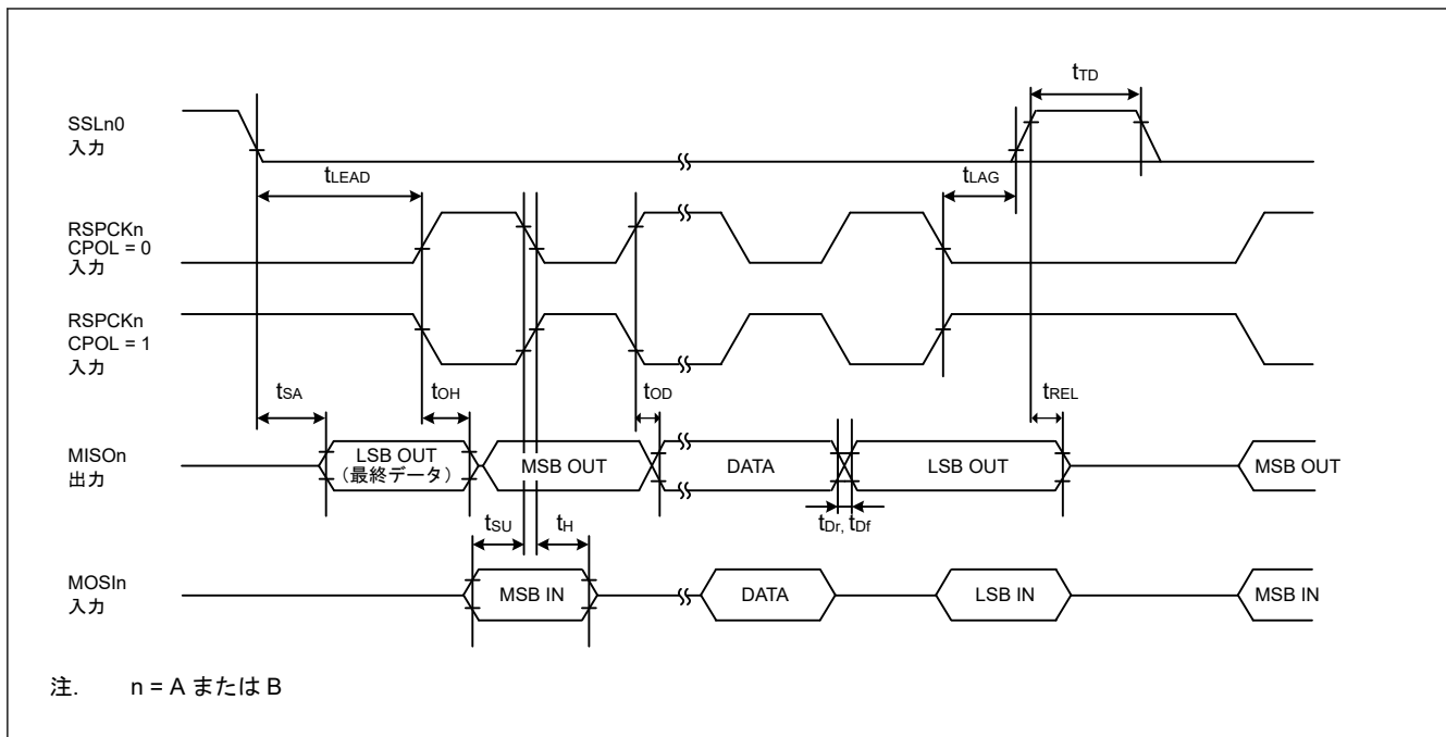
図 41.40 CPHA = 1 の場合におけるスレーブの SPI タイミング
