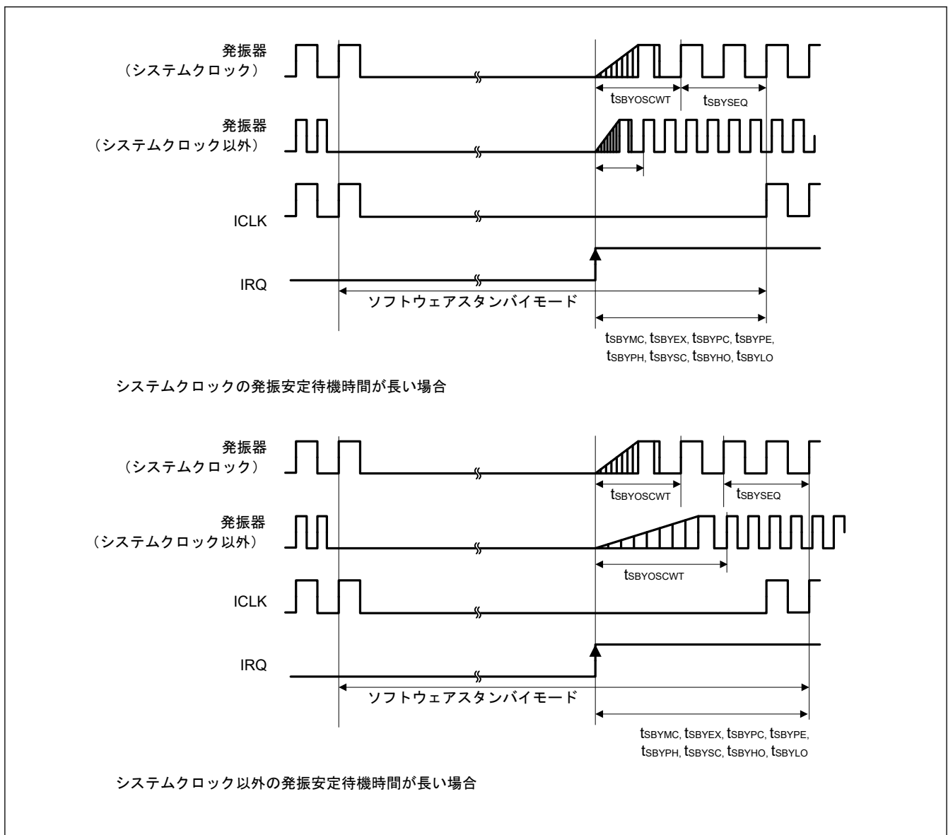
図 41.14 ソフトウェアスタンバイモード解除タイミング
