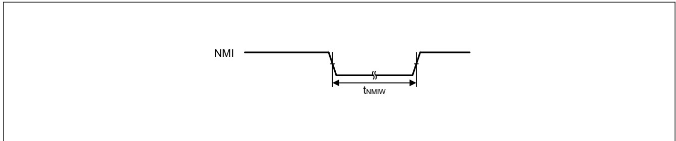
図 41.17 NMI 割り込み入力タイミング
