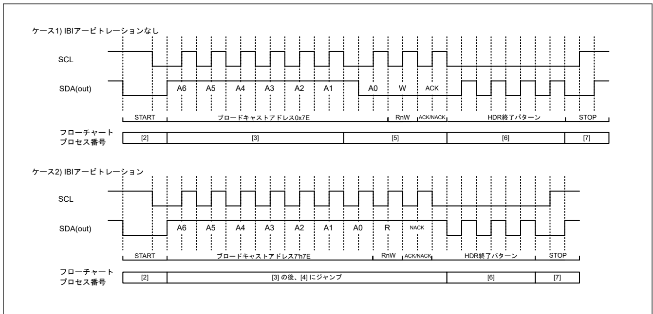
図 25.98 I3C マスタの I3C エスカレーション処理タイミングチャート
