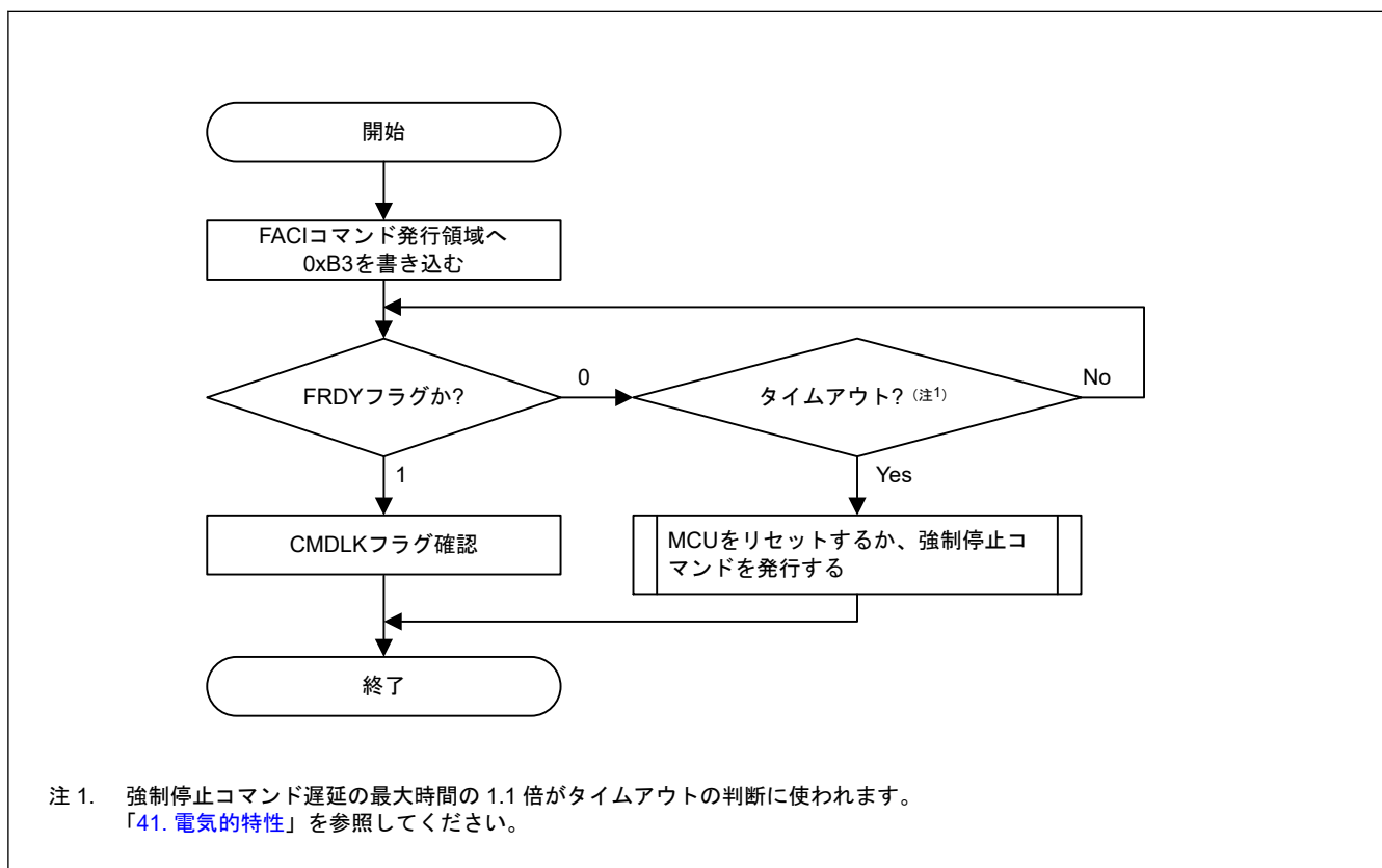
図 38.22 強制停止コマンドの使用フロー
