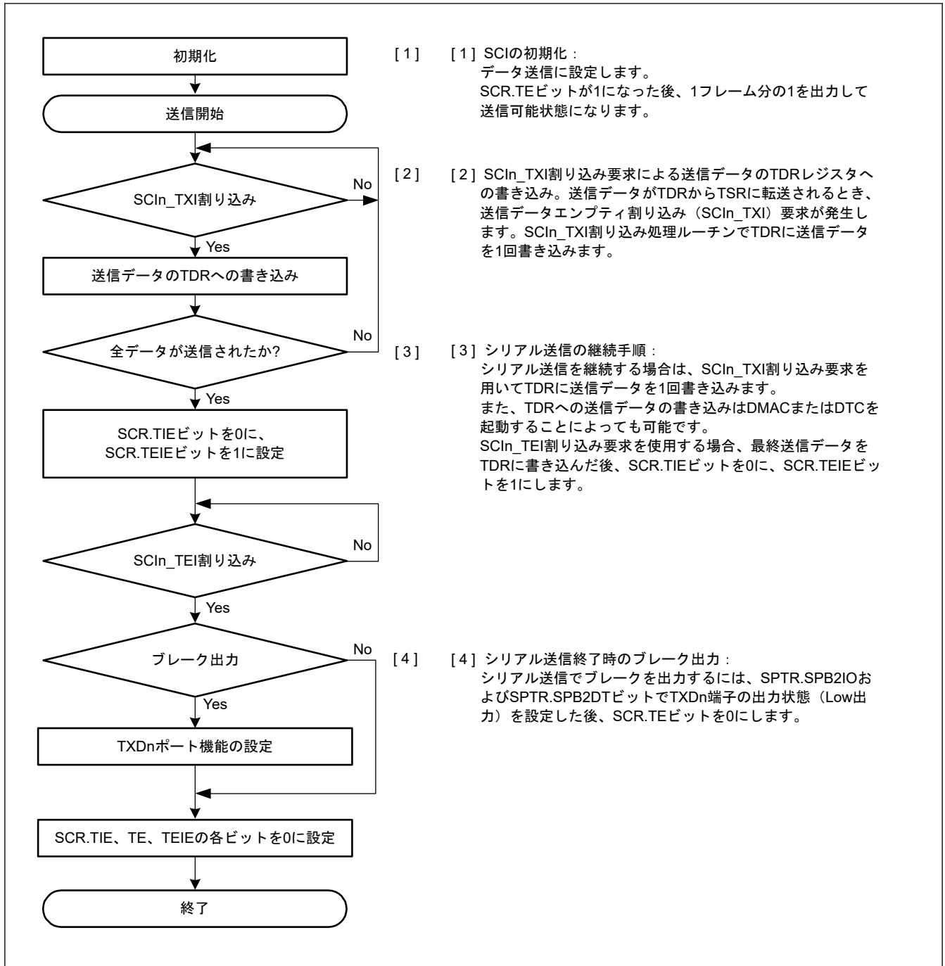
図 24.12 調歩同期式モードにおけるシリアル送信のフローチャート例 (非 FIFO 選択時)
