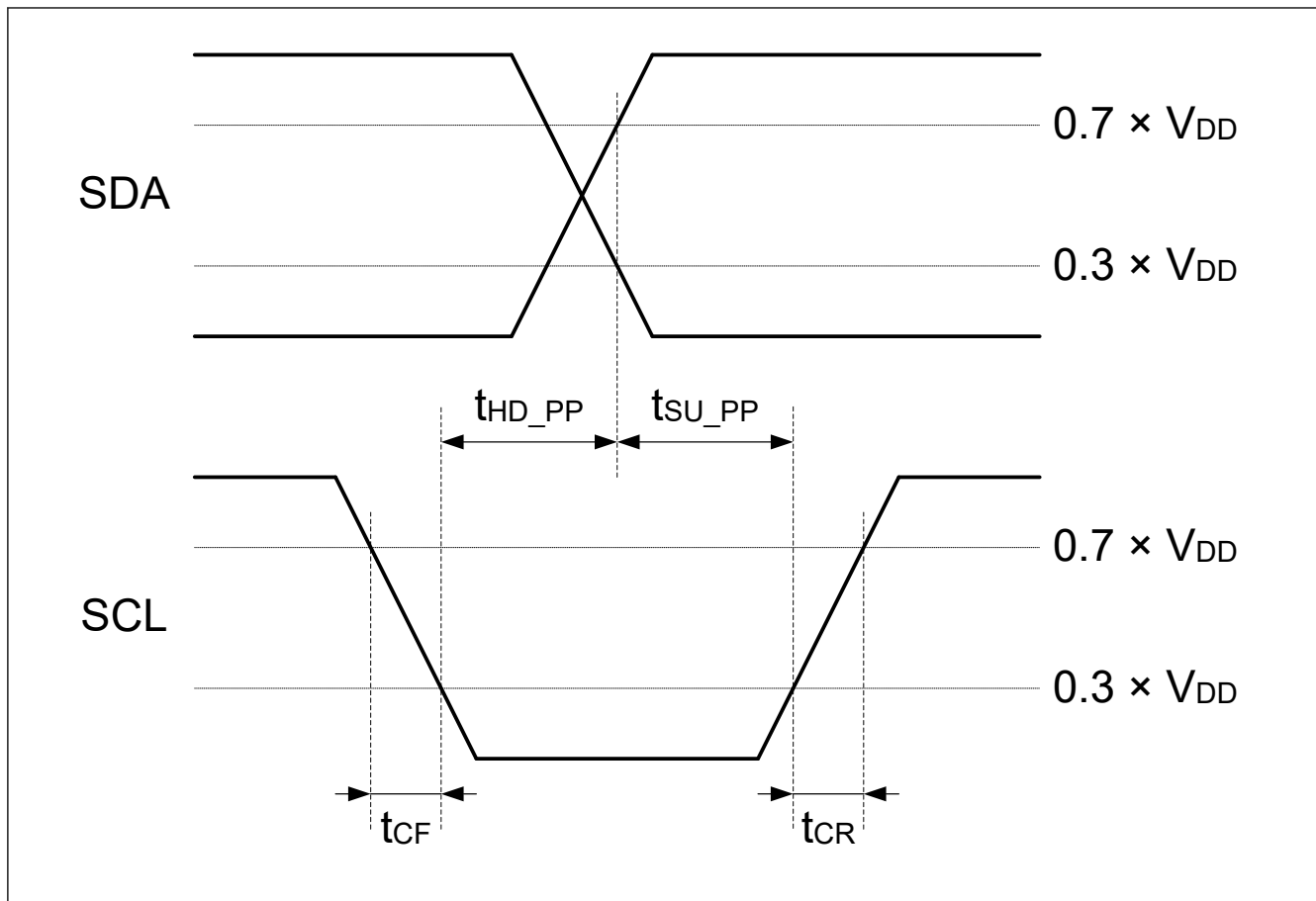
図 41.47 I3C マスタ出カタイミング
