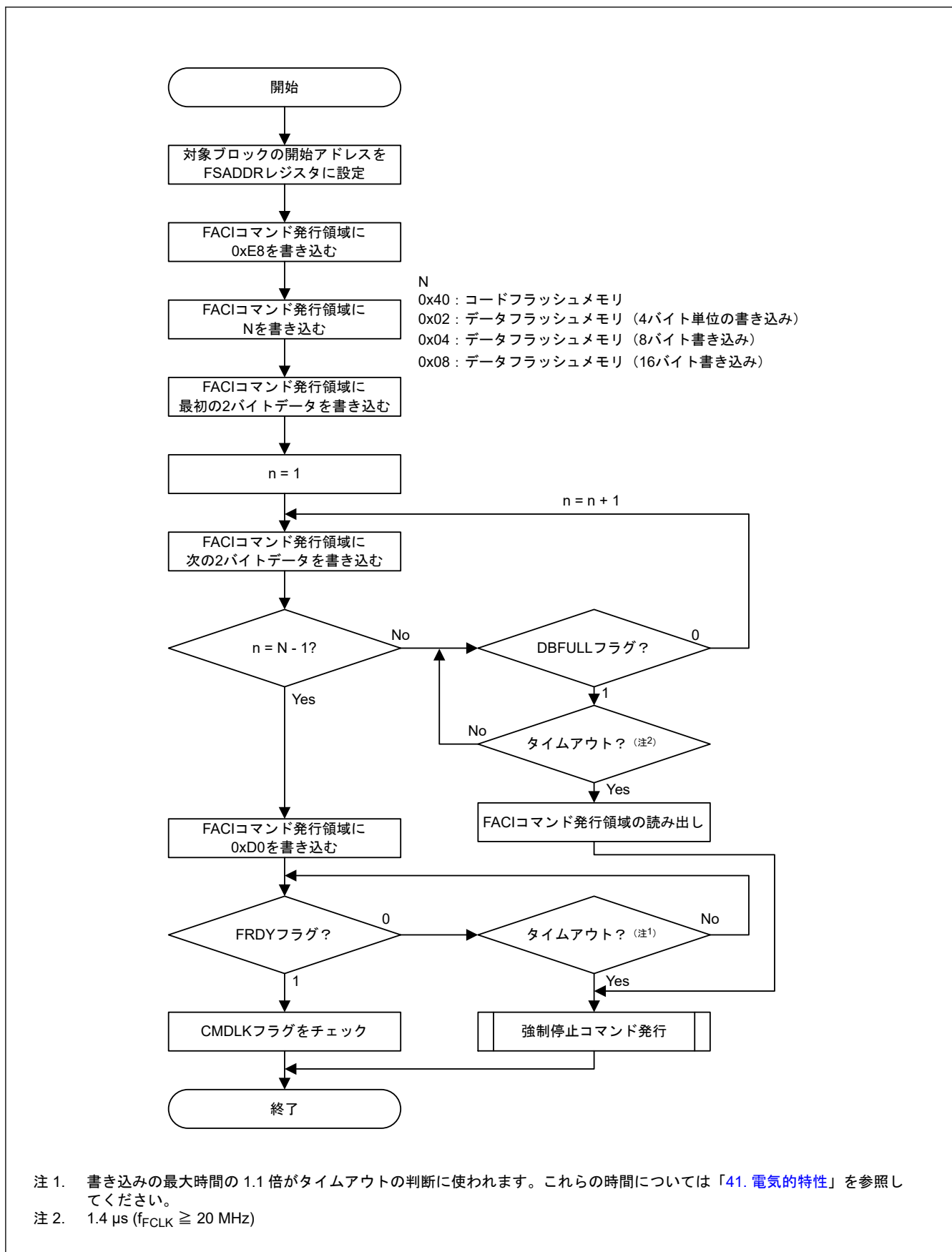
図 38.13 プログラムコマンドの使用フロー
