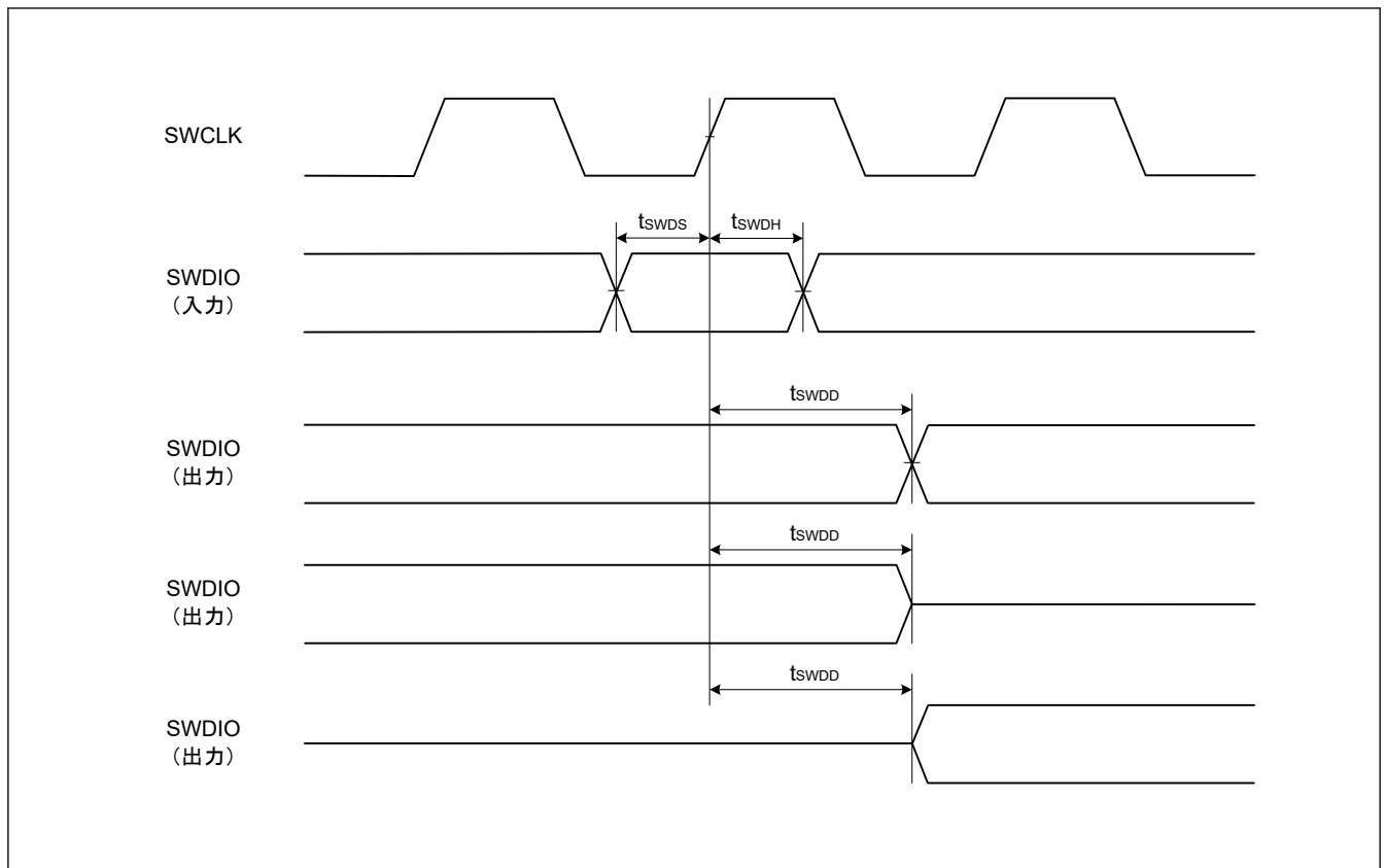
図 41.61 SWD 入出力タイミング
