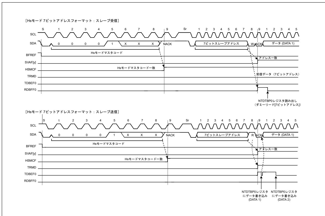
図 25.65 Hs モードマスターコード受信時に SVAF[y]、HSMCF フラグが 1 になるタイミング
