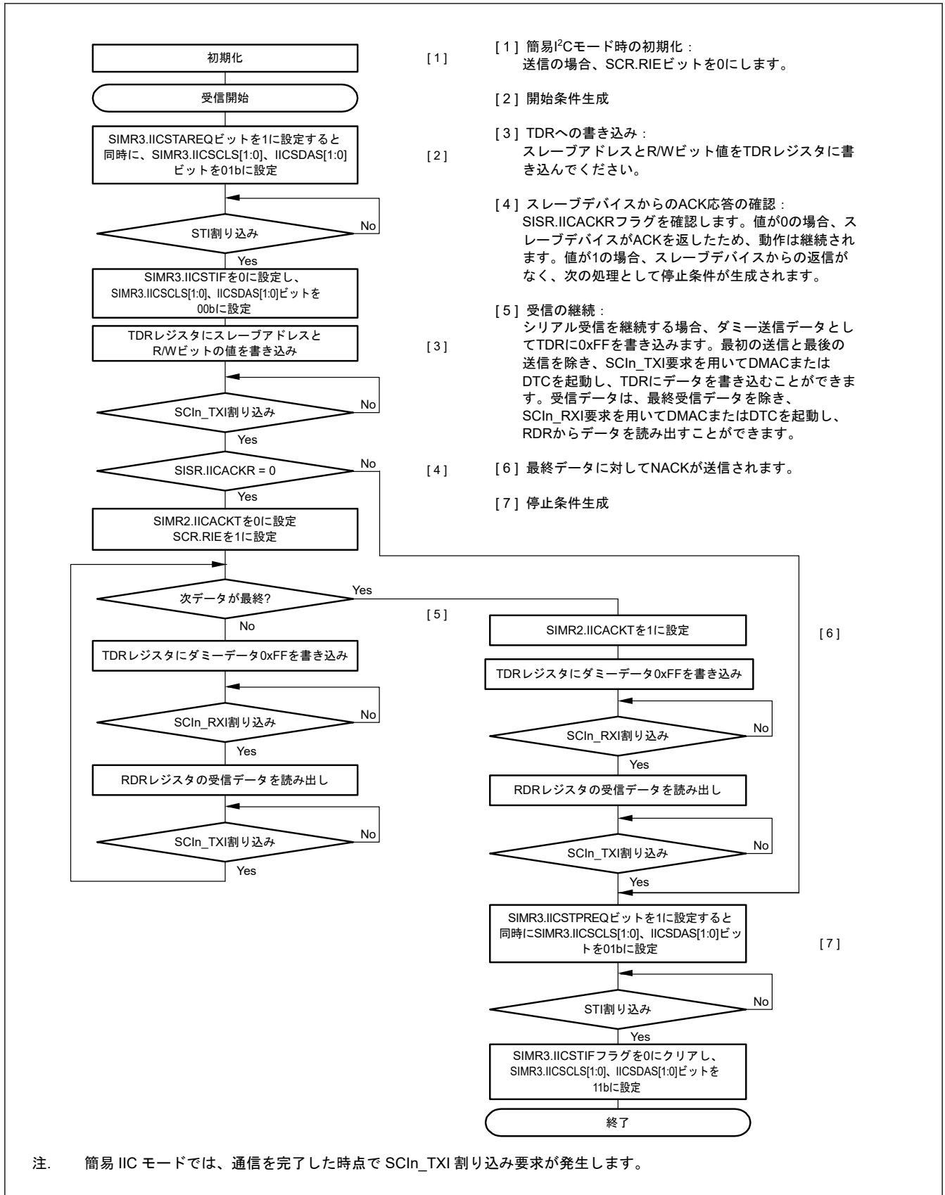
図 24.94 簡易 IIC モードにおけるマスタ受信のフローチャート例（送信割り込み、受信割り込み使用時）
