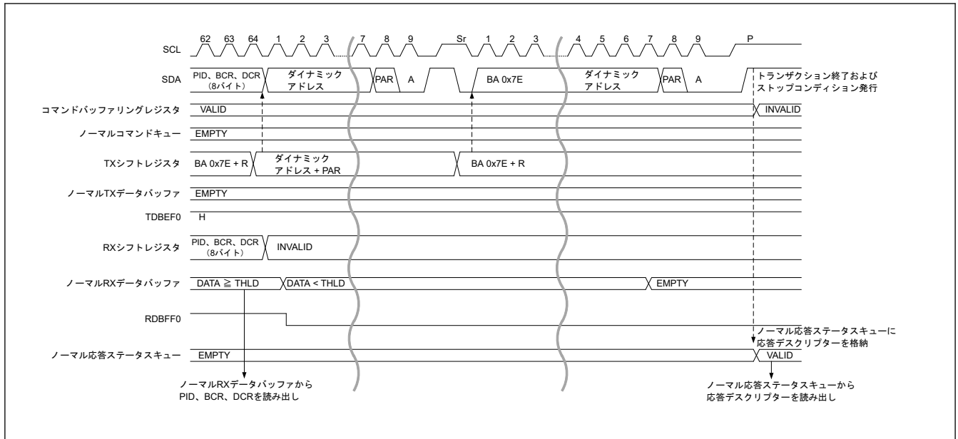
図 25.14 ダイナミックアドレス配置手順 (ENTDAACCC) タイミング (3/3)
