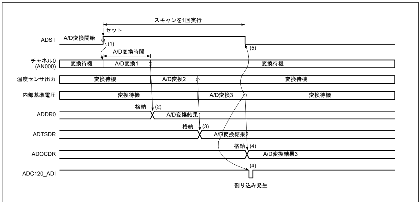
図 32.13 シングルスキャンモードの基本動作例 (AN000、温度センサ出力または内部基準電圧選択時)
