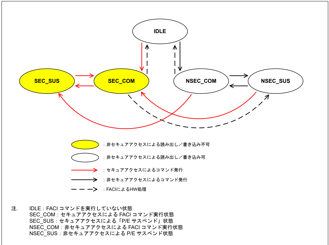
図 38.33 FACL コマンド動作中の保護状態
