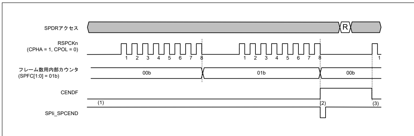
図 30.45 通信終了割り込み動作例 (クロック同期式動作時の受信のみスレーブモード)
