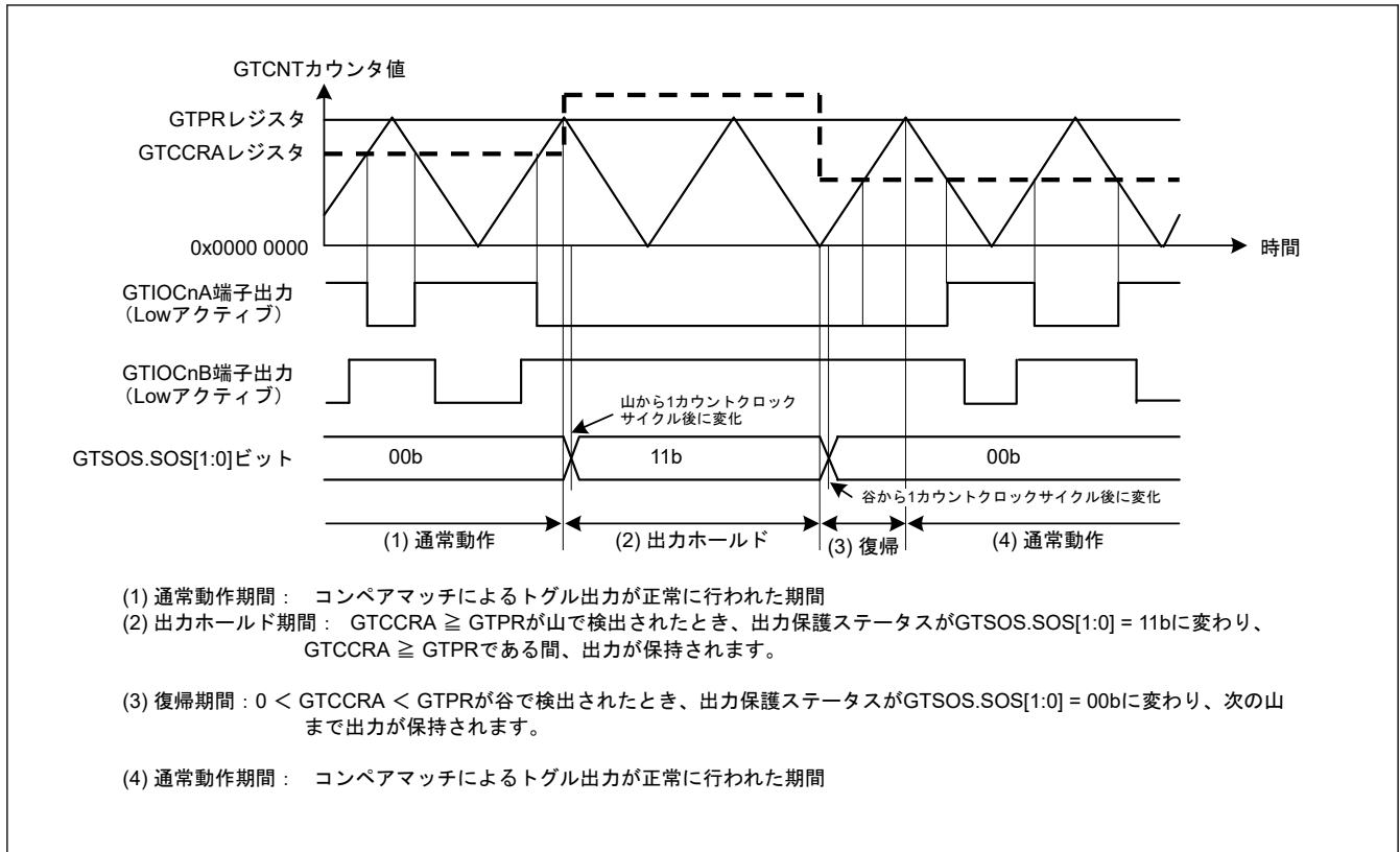
図 21.180 山のバッファ転送で GTCCRA レジスタ \geq GTPR レジスタとなった場合の出力保護機能の動作例 (谷のバッファ転送で 0 < GTCCRA レジスタ < GTPR レジスタに復帰、アクティブレベルは Low の場合) (n = 0~9)
