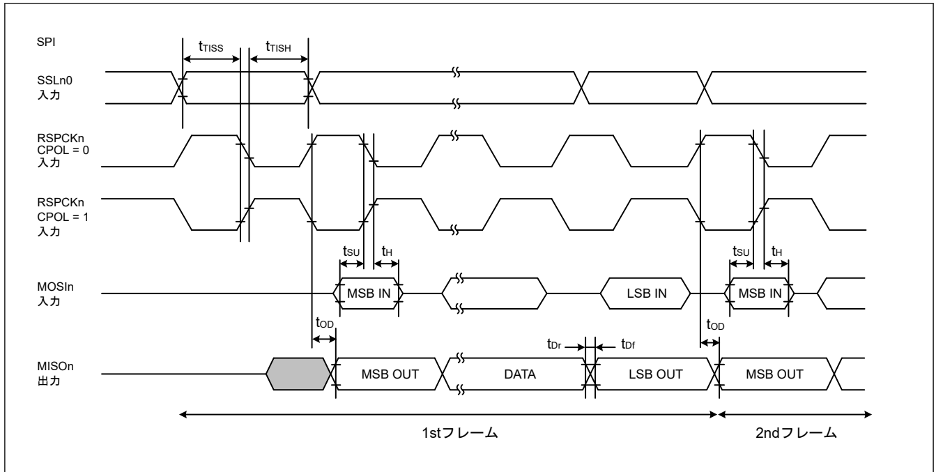
図 46.46 フレーム間の遅延がない送信における TI SSP スレーブの SPI タイミング
