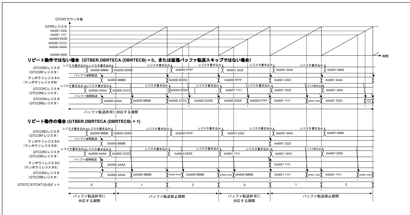
図 21.167 GTCCR バッファ転送禁止時のリピートダブルバッファ動作例 (のこぎり波ワンショットパルスモード、拡張バッファ転送スキップ機能使用、GTBER.BD[0]ビットが常に0の場合)
