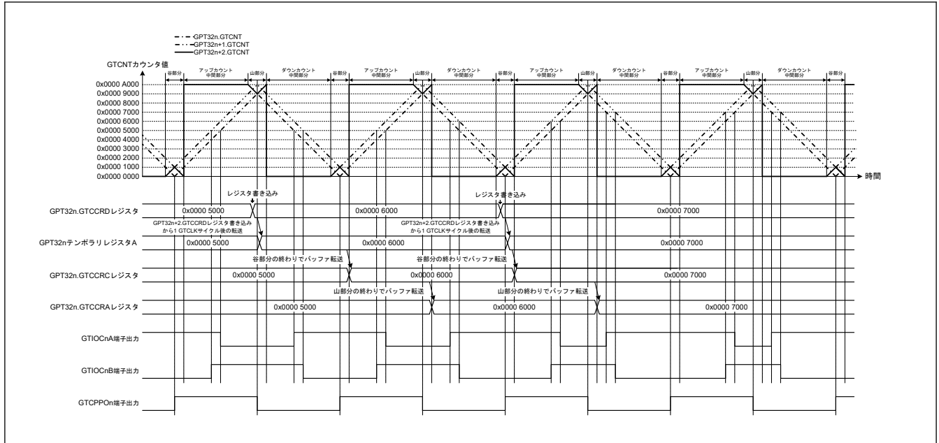
図 21.49 相補 PWM モード 1 動作例 (アップカウントの GTCCRA レジスタコンペアマッチ時 : GTIOCnA 端子 = Low/GTIOCnB 端子 = High、ダウンカウントの GTCCRA レジスタコンペアマッチ時 : GTIOCnA 端子 = High/GTIOCnB 端子 = Low、デッドタイム値 : 0x0000 1000、GTCCRD レジスタを山部分と谷部分で更新) (n = 4、7)
