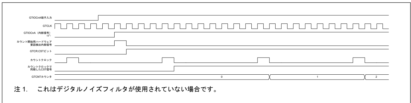
図 21.88 GTIOcNA 端子の入力の立ち上がりエッジに対応するカウントスタート動作のタイミング例
