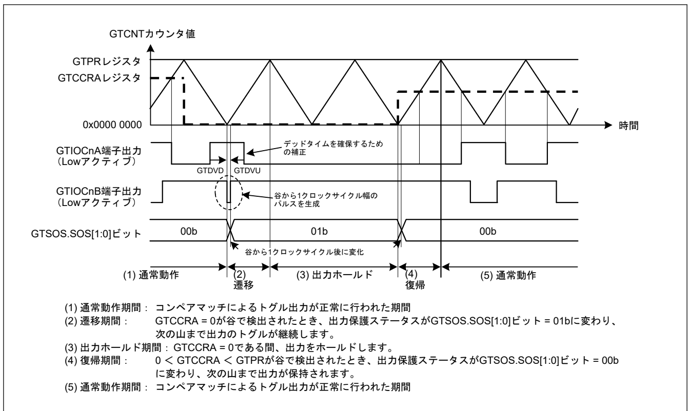
図 21.175 谷のバッファ転送で GTCRA レジスタが 0x0000 0000 である場合の出力保護機能の動作例 (山のバッファ転送で 0 < GTCRA レジスタ < GTPR レジスタに復帰、アクティブレベルは Low の場合) ( n = 0 \sim 9 )
