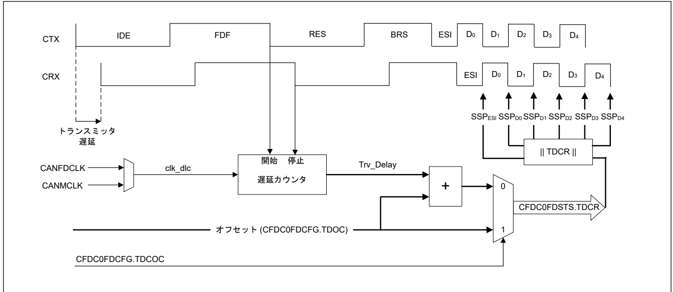
図 28.18 トランスミッタ遅延補償
