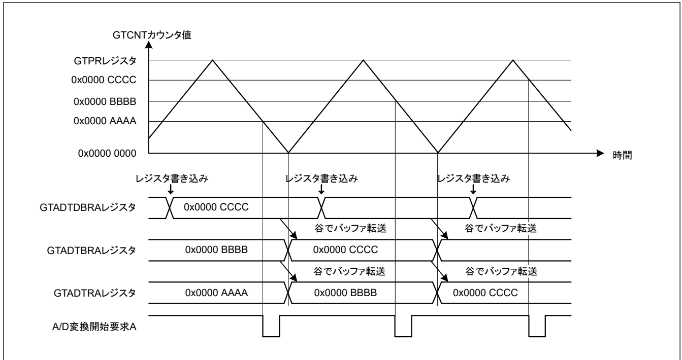
図 21.33 GTADTRA、GTADTRB レジスタのダブルバッファ動作例（三角波、谷でバッファ転送、ダウンカウントで A/D 変換開始要求発生の場合）
