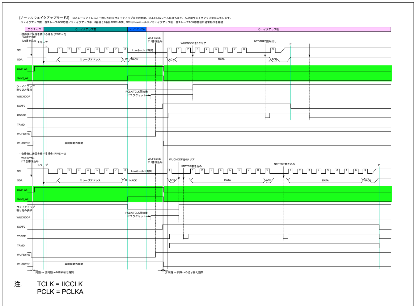
図 27.39 ノーマル WU モード 2 のタイミング
