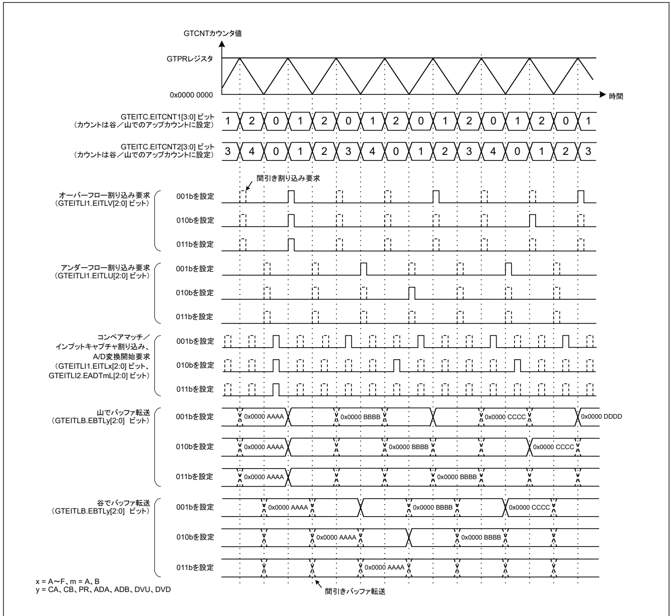
図 21.152 拡張割り込み間引き機能の動作例 (三角波、山と谷の両方をカウント、拡張割り込み間引き 1 の間引き回数は 2 回、山と谷の両方をカウント、拡張割り込み間引き 2 の間引き回数は 4 回、拡張割り込み間引きカウンタ 2 の初期値は 0、GTEITC.EITCNTk ビット (k = 1, 2) が 0 以外の期間に間引く場合)
