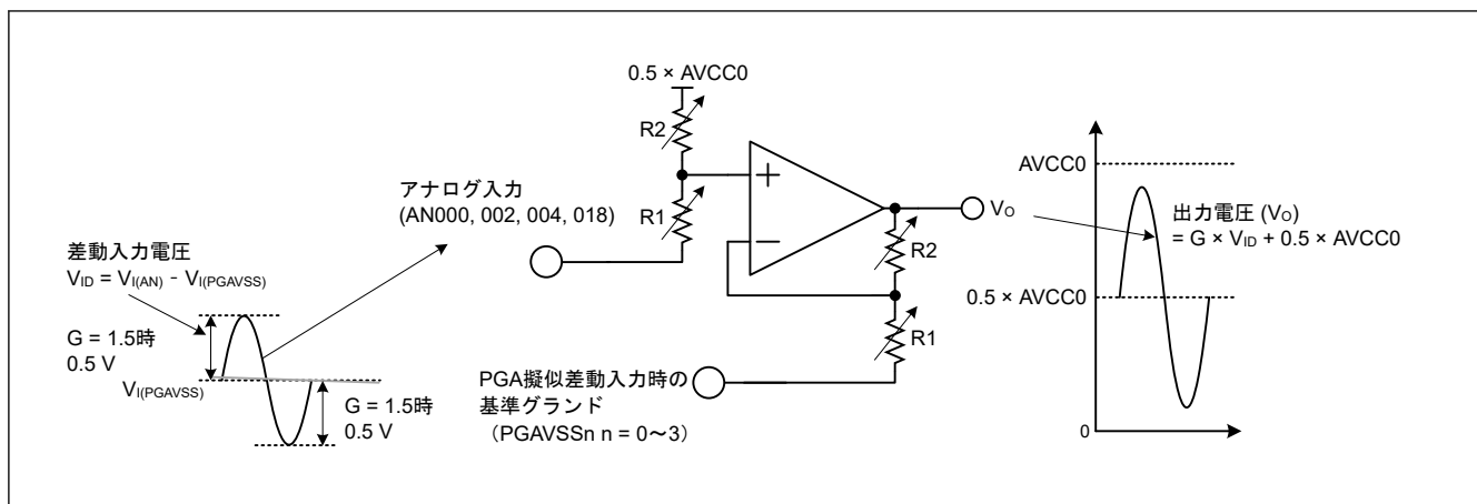
図 46.53 PGA 疑似差動設定時の入出力信号レベル
