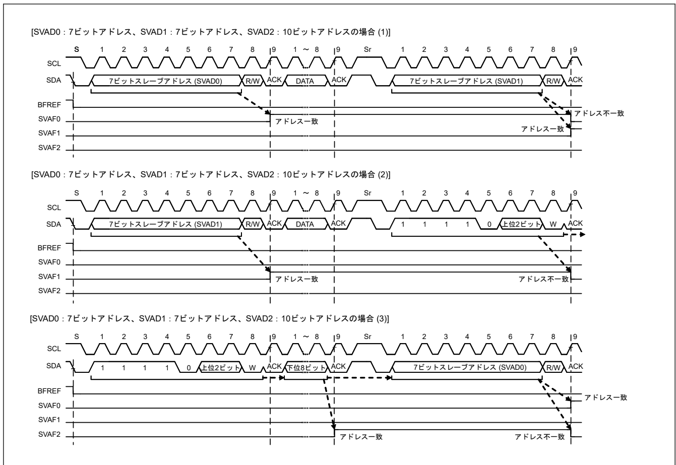
図 27.20 SDAFy フラグが 1 または 0 になるタイミング (7 ビット/10 ビットアドレスフォーマット混在時)
