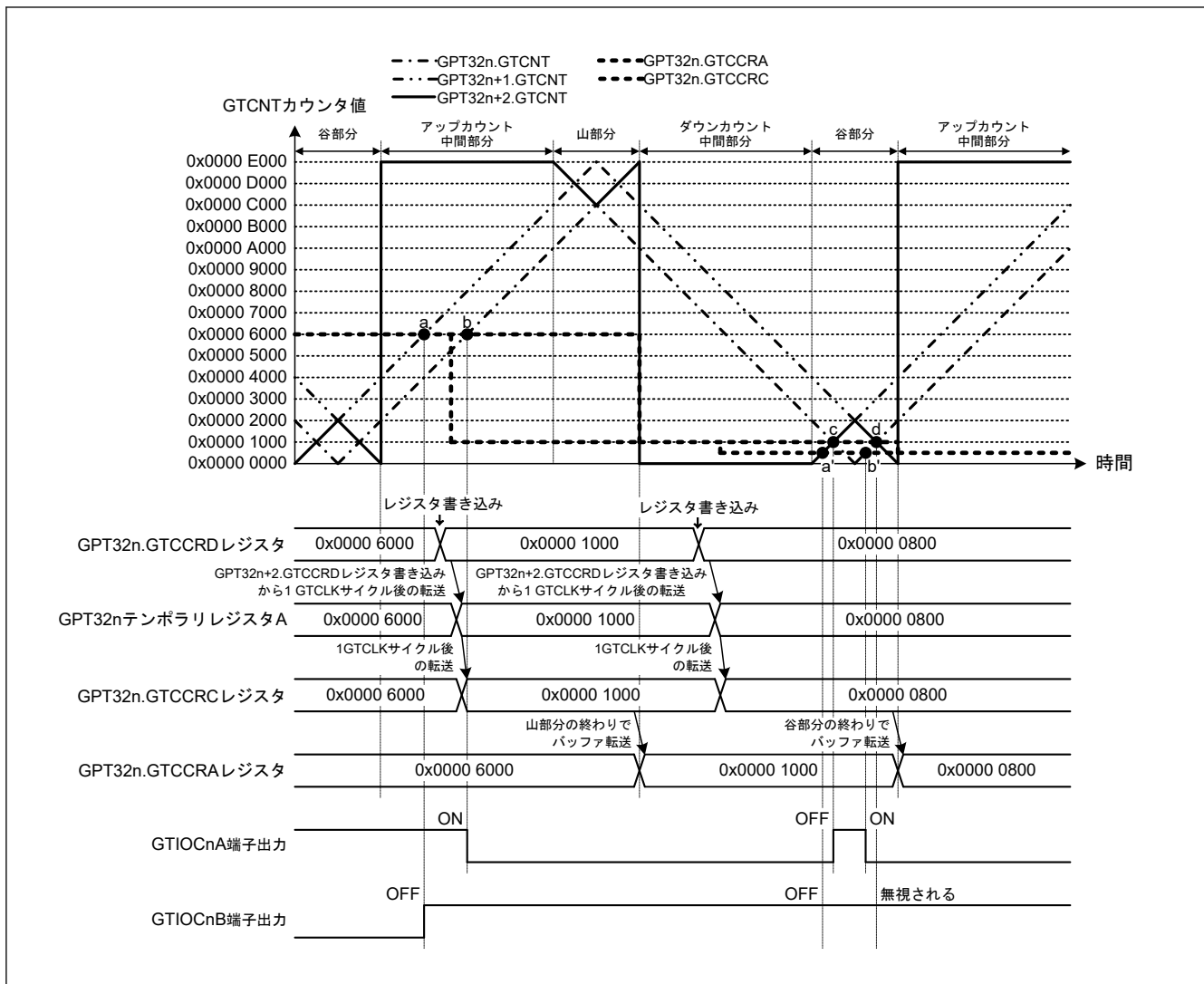
図 21.66 相補 PWM モードでのコンペアマッチ発生シーケンス動作例 (相補 PWM モード 3 シングルバッファ動作、アップカウントの GTCCRA レジスタコンペアマッチ時 : GTIOCnA 端子 = Low / GTIOCnB 端子 = High、ダウンカウントの GTCCRA レジスタコンペアマッチ時 : GTIOCnA 端子 = High / GTIOCnB 端子 = Low、デッドタイム値 : 0x0000 2000、コンペアマッチ発生順序 : a' → c → b' → d) (n = 4, 7)
