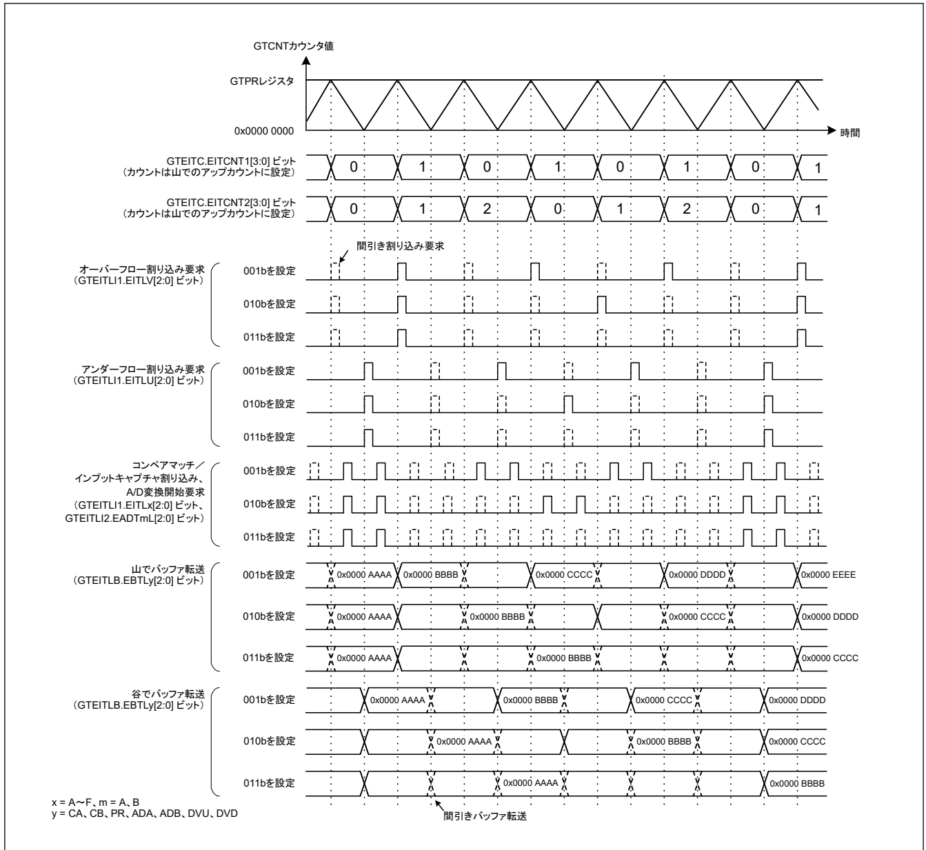
図 21.150 拡張割り込み間引き機能の動作例 (三角波、山をカウント、拡張割り込み間引き 1 の間引き回数は 1 回、山をカウント、拡張割り込み間引き 2 の間引き回数は 2 回、拡張割り込み間引きカウンタ 2 の初期値は 0、GTEITC.EITCNTk ビット (k = 1, 2) が 0 以外の期間に間引く場合)
