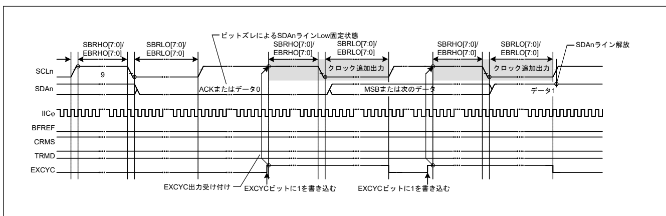
図 27.32 SCL クロック追加出力機能 (EXCYC ビット)
