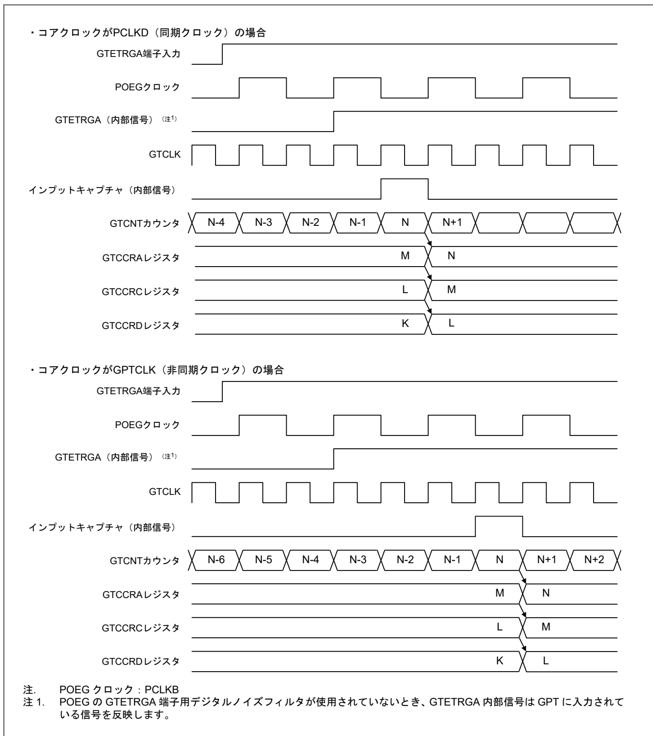
図 21.15 GTETRGA 端子の入力の立ち上がりエッジに対応するインプットキャプチャ動作のタイミング例
