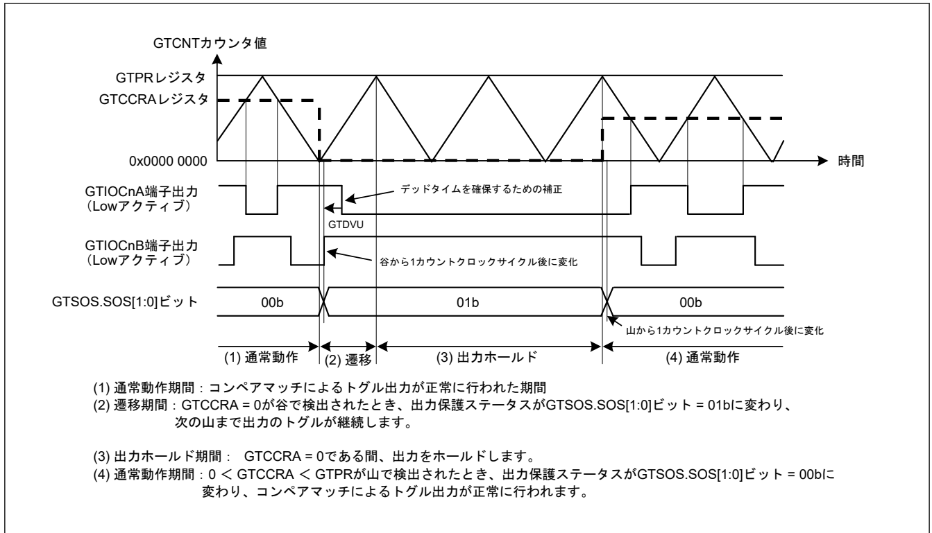
図 21.174 谷のバッファ転送で GTCRA レジスタが 0x0000 0000 である場合の出力保護機能の動作例 (山のバッファ転送で 0 < GTCRA レジスタ < GTPR レジスタに復帰、アクティブレベルは Low の場合) ( n = 0 \sim 9 )
