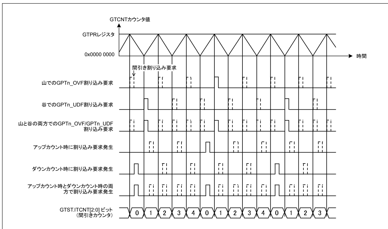
図 21.142 割り込み間引き機能の動作例（三角波、谷と山の両方をカウントして間引き、間引き回数 4 の場合）
