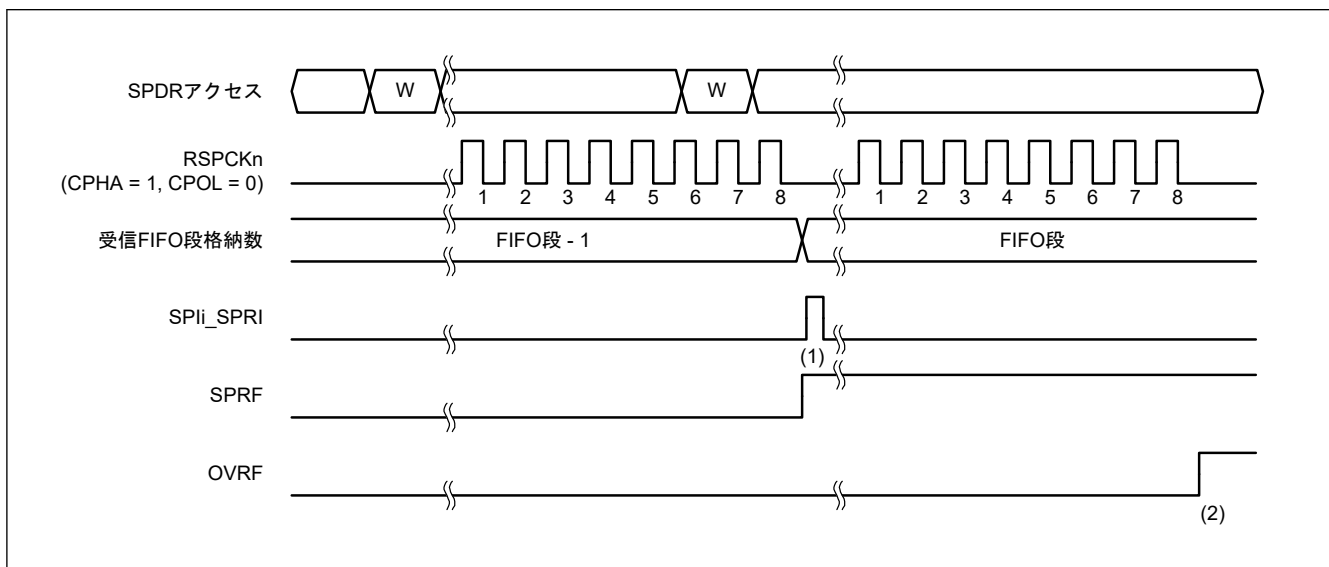
図 30.30 SPCR.TXMD[1:0] = 00b の動作例
