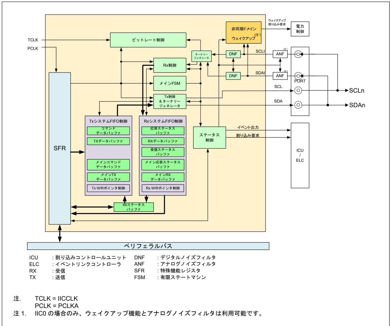
図 27.1 IIC ブロック図
