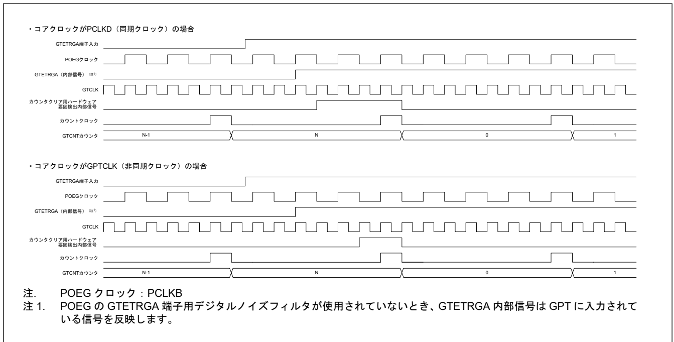
図 21.98 GTETRGA 端子入力の立ち上がりエッジに対応するカウンタクリアの動作タイミング例 (GTCLK 信号の分周により生成されるクロック信号の周期計数中)
