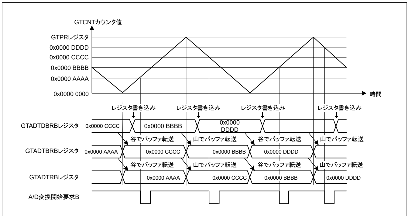
図 21.34 GTADTRA、GTADTRB レジスタのダブルバッファ動作例（三角波、谷と山の両方でバッファ転送、アップカウントとダウンカウントの両方で A/D 変換開始要求発生の場合）
