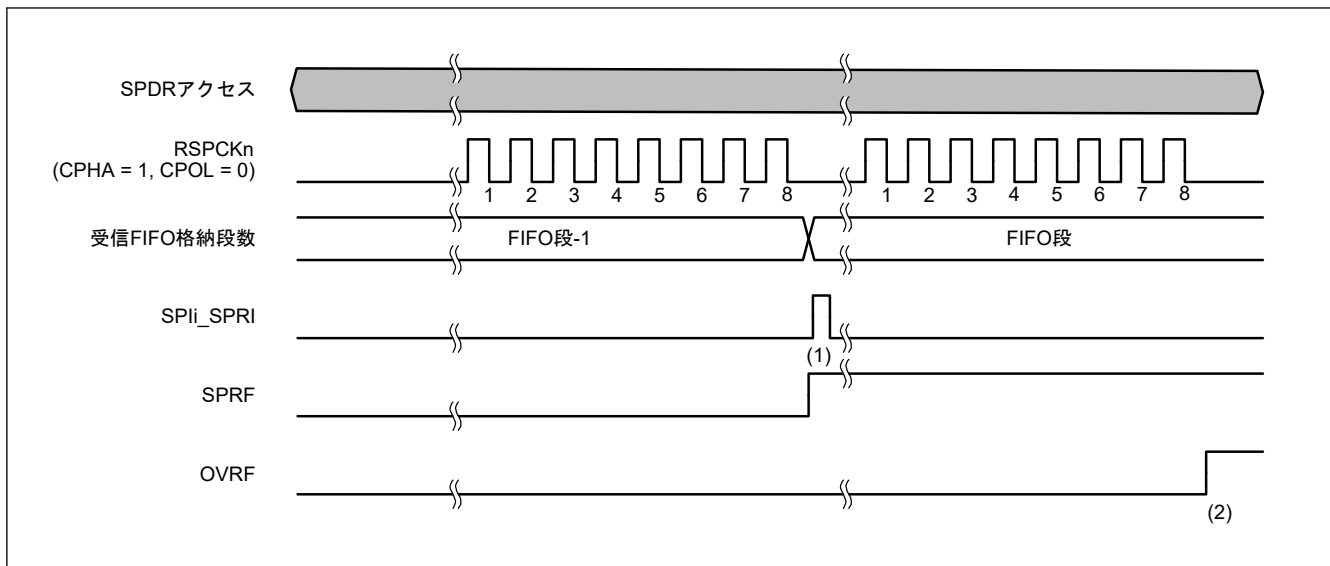
図 30.32 SPCR.TXMD[1:0] = 10b の場合の動作例
