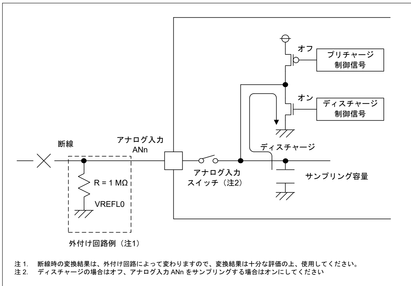
図 36.25 ディスチャージを選択した場合の断線検出例
