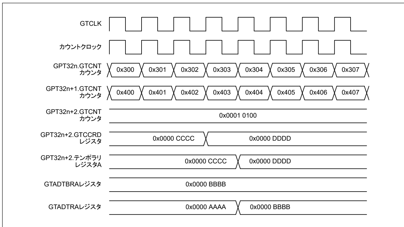
図 21.35 相補 PWM モードでのスレーブチャンネル 2 の GTCCRD レジスタ更新の場合の GTADTRA、GTADTRB レジスタのバッファ動作例
