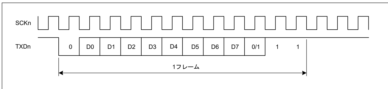
図 26.6 調歩同期式モードにおける出力クロックと送信データの位相関係 (CCR1.PE = 1、CCR3.CHR[1:0] = 10b、MP = 0、および STP = 1 の場合)
