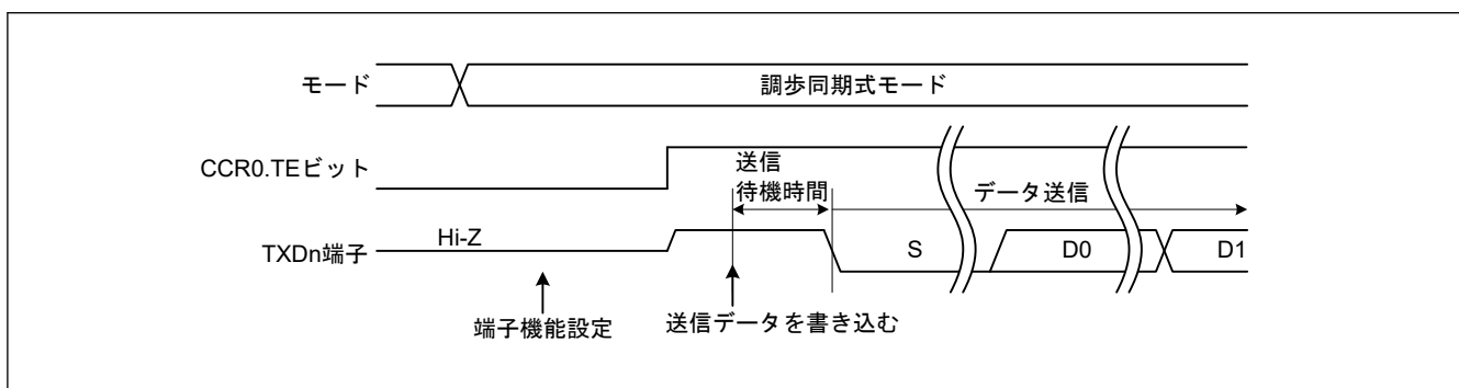
図 26.9 調歩同期モードでのデータ送信タイミング例
