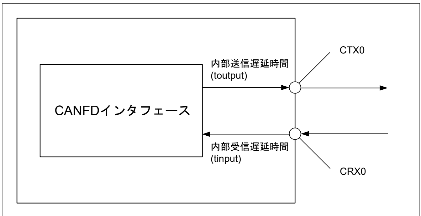
図 46.49 CANFD インタフェース条件
