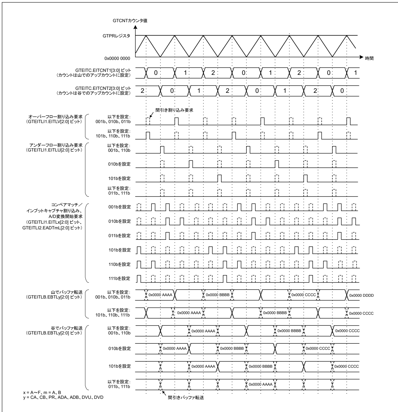
図 21.148 拡張割り込み間引き機能の例 (三角波、山をカウント、拡張割り込み間引き 1 の間引き回数は 2 回、谷をカウント、拡張割り込み間引き 2 の間引き回数は 2 回、拡張割り込み間引きカウンタ 2 の初期値は 0 の場合)
