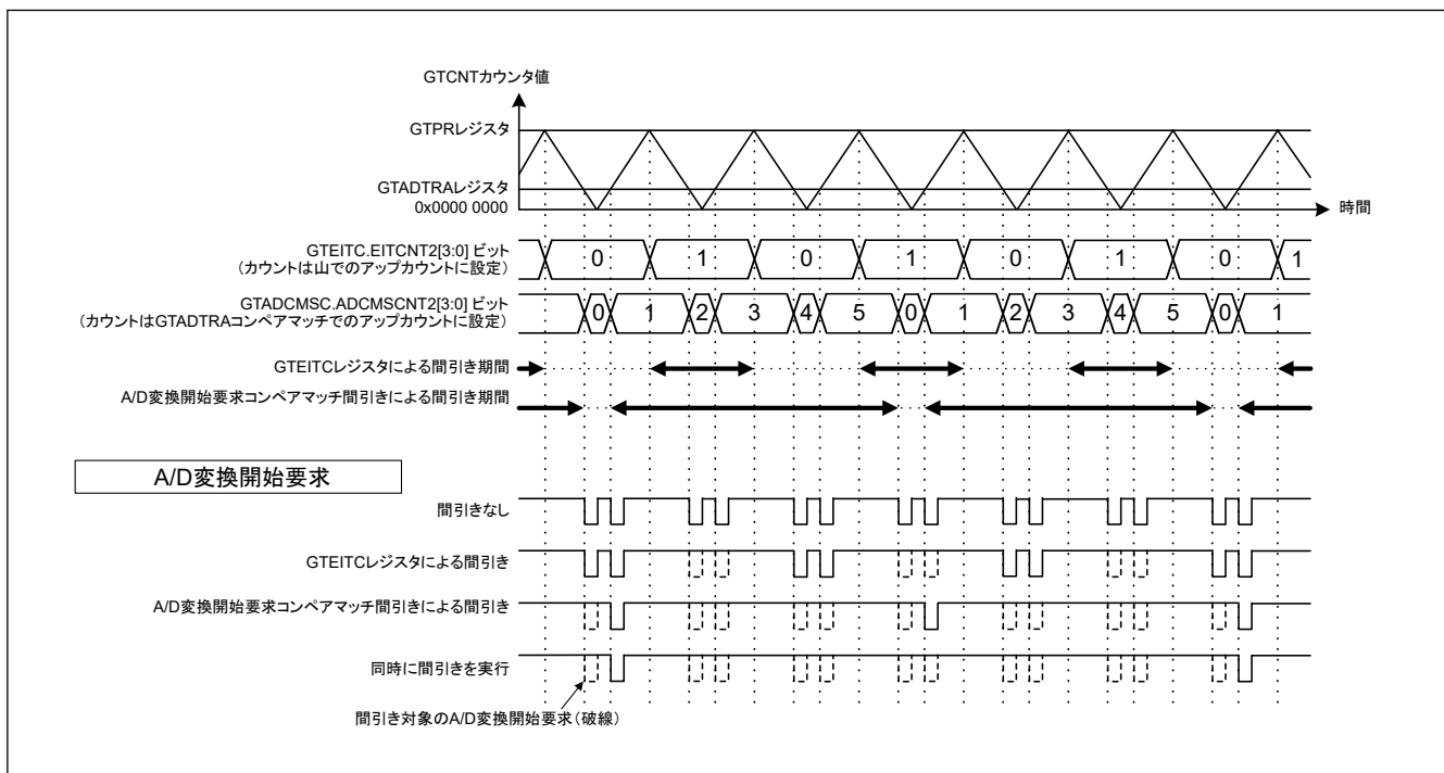
図 21.158 A/D 変換開始要求コンペアマッチ間引き機能の動作例 (拡張割り込み間引き : EIVTC2[1:0] = 01b、EADTAL[2:0] = 010b、A/D 変換開始要求コンペアマッチ間引き : ADCMS2[1:0] = 01b、ADCMSAL[2:0] = 010b の場合)
