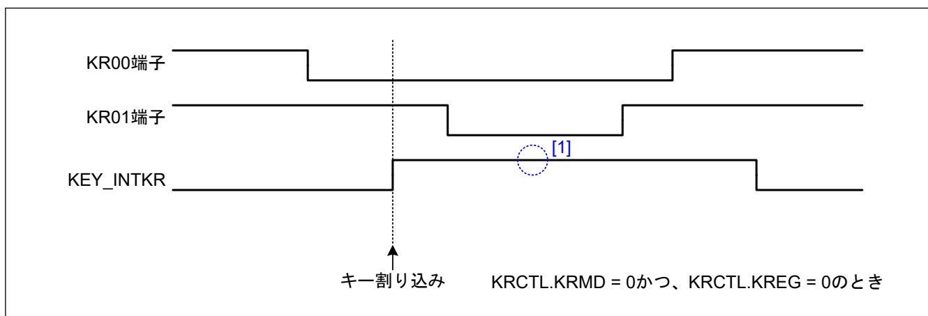
図 19.3 キー割り込みが複数のチャンネルに入力された場合の KEY_INTKR 信号の動作
