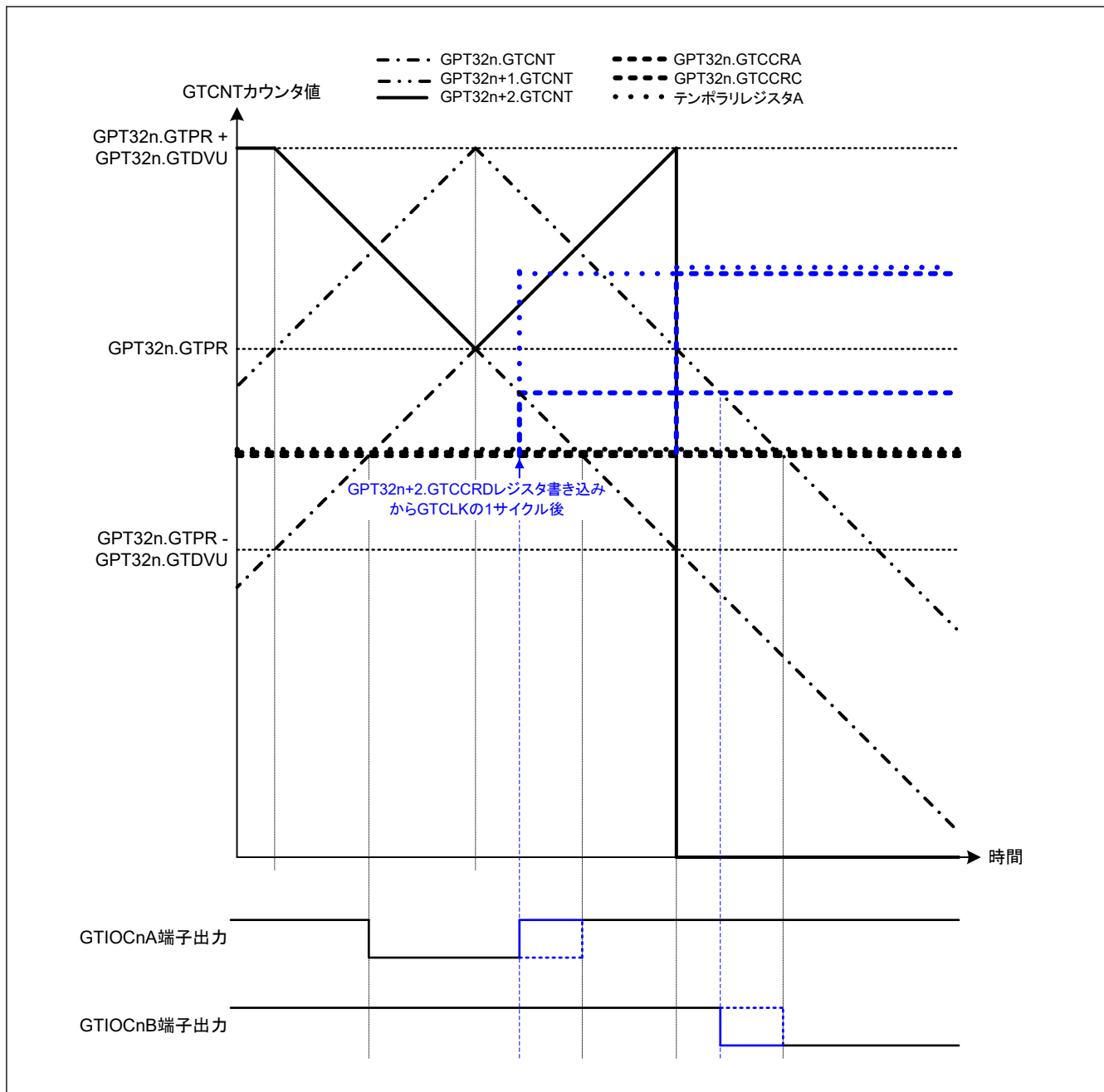
図 21.73 相補 PWM モード 4 でのシングルバッファ動作例 (ダウンカウント山部分) (相補 PWM モード 4 のシングルバッファ動作、アップカウントの GTCCRA レジスタコンペアマッチ時: GTIOCN A 端子 = Low / GTIOCN B 端子 = High、ダウンカウントの GTCCRA レジスタコンペアマッチ時: GTIOCN A 端子 = High / GTIOCN B 端子 = Low、アップカウントのコンペアマッチ後でダウンカウントのコンペアマッチ前に GPT32n.GTCNT 値以上の値を GTCCRD レジスタに書き込んだ場合) (n = 4, 7)
