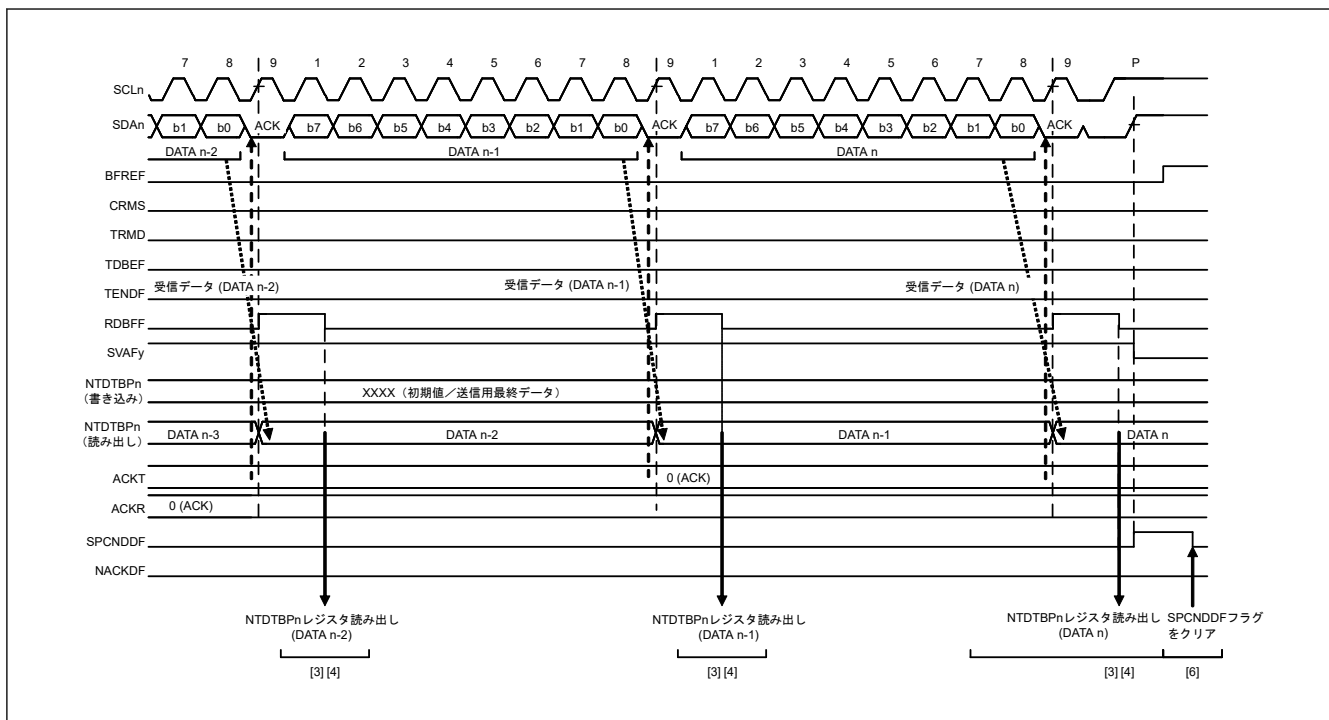
図 27.9 スレーブ受信の動作タイミング (2) (ACKTWE = 0 の場合)
