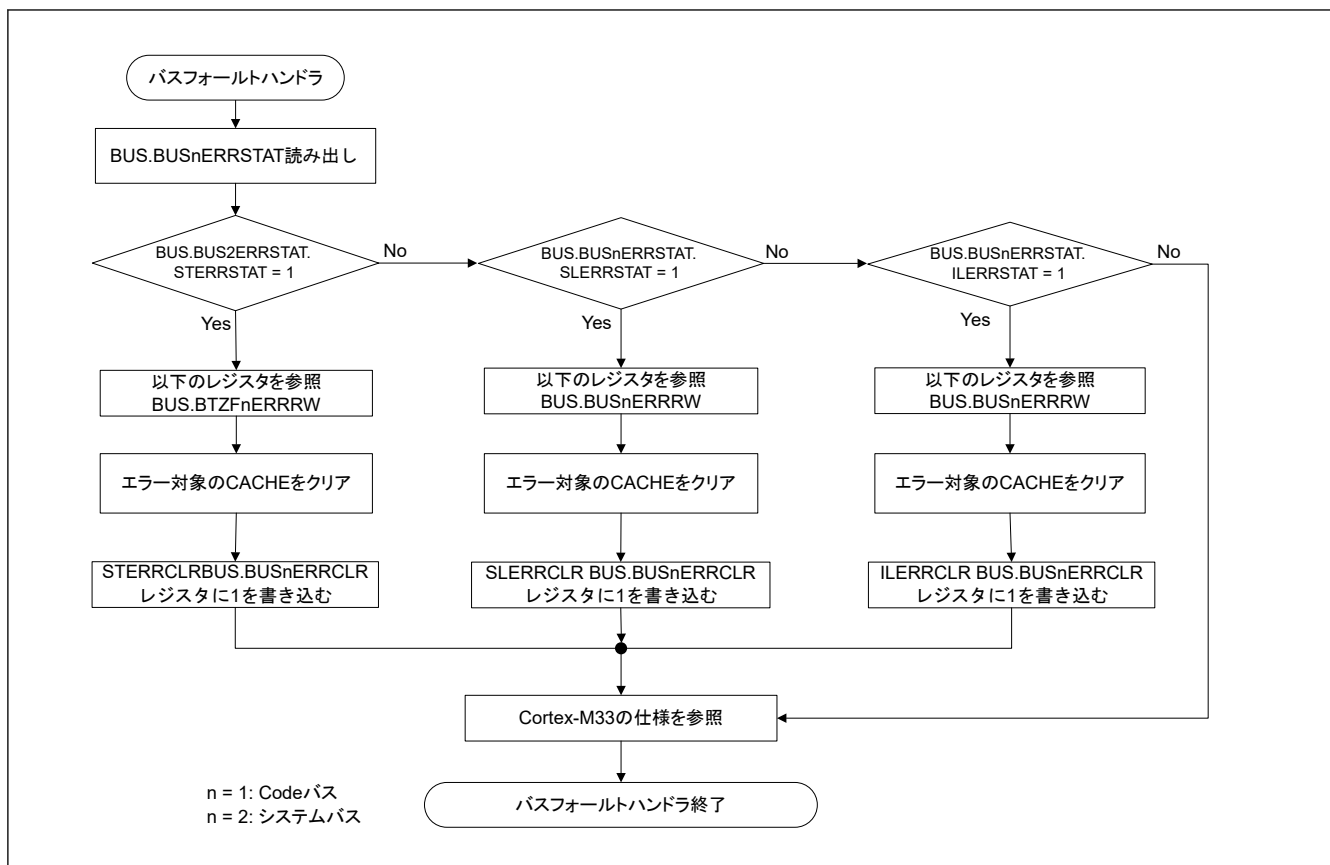
図 2.5 バスフォールト割り込み処理フローチャート
