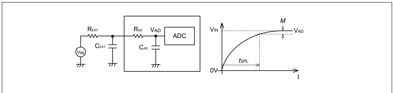
図 36.60 A/D コンバータのサンプル&ホールド回路の簡略図
