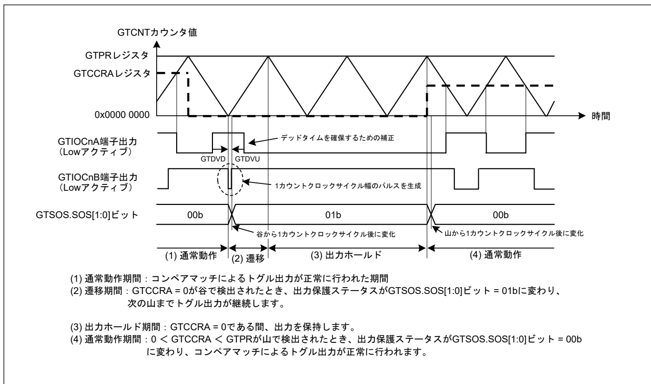
図 21.176 山のバッファ転送で GTCRA レジスタが 0x0000 0000 である場合の出力保護機能の動作例 (山のバッファ転送で 0 < \text{GTCRA レジスタ} < \text{GTPR レジスタ} に復帰、アクティブレベルは Low の場合) ( n = 0 \sim 9 )
