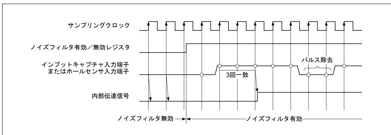
図 21.163 ノイズフィルタのタイミング
