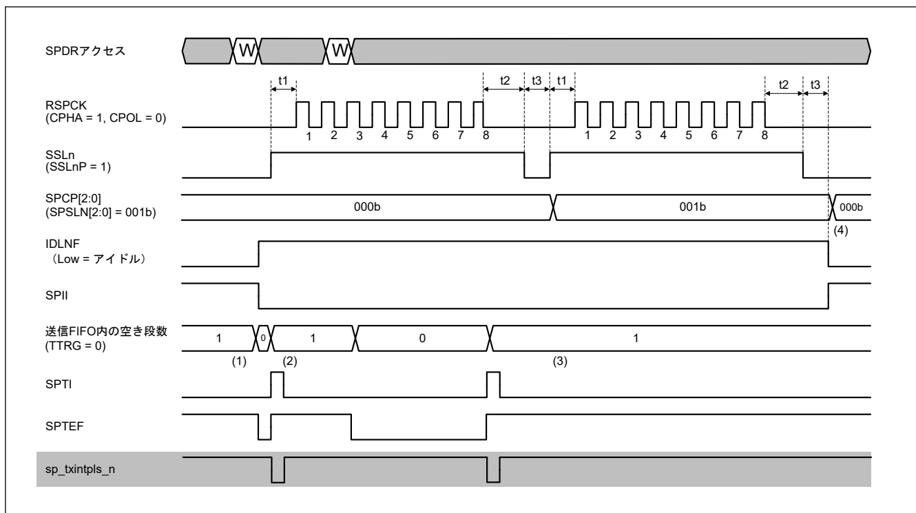
図 30.34 アイドル割り込み動作の例 (マスタモード/Motorola-SPI)
