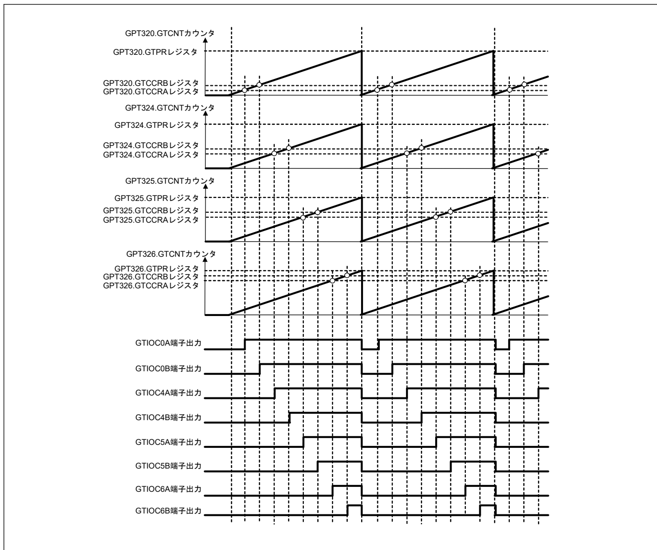
図 21.112 同期 PWM 出力例
