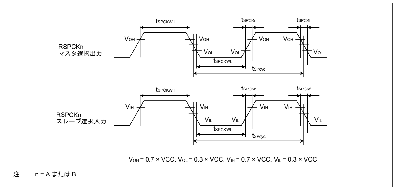
図 46.39 SPI クロックタイミング
