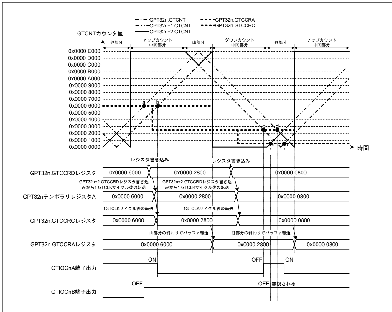
図 21.64 相補 PWM モードでのコンペアマッチ発生シーケンス動作例 (相補 PWM モード 3 シングルバッファ動作、アップカウントの GTCCRA レジスタコンペアマッチ時 : GTIOCnA 端子 = Low/GTIOCnB 端子 = High、ダウンカウントの GTCCRA レジスタコンペアマッチ時 : GTIOCnA 端子 = High/GTIOCnB 端子 = Low、デッドタイム値 : 0x0000 2000、コンペアマッチ発生順序 : c → a' → d → b') (n = 4, 7)
