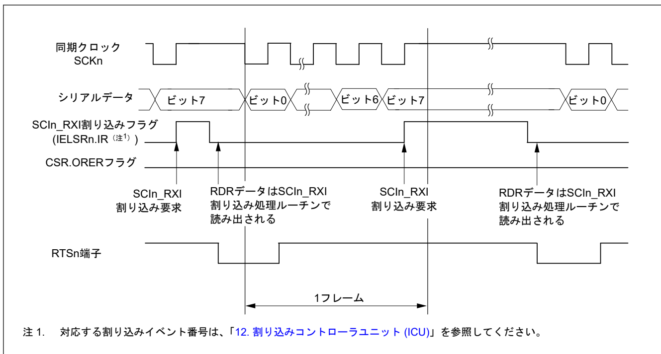
図 26.66 クロック同期式モードにおけるシリアル受信の動作例 (2) (RTS 機能を使用する場合)
