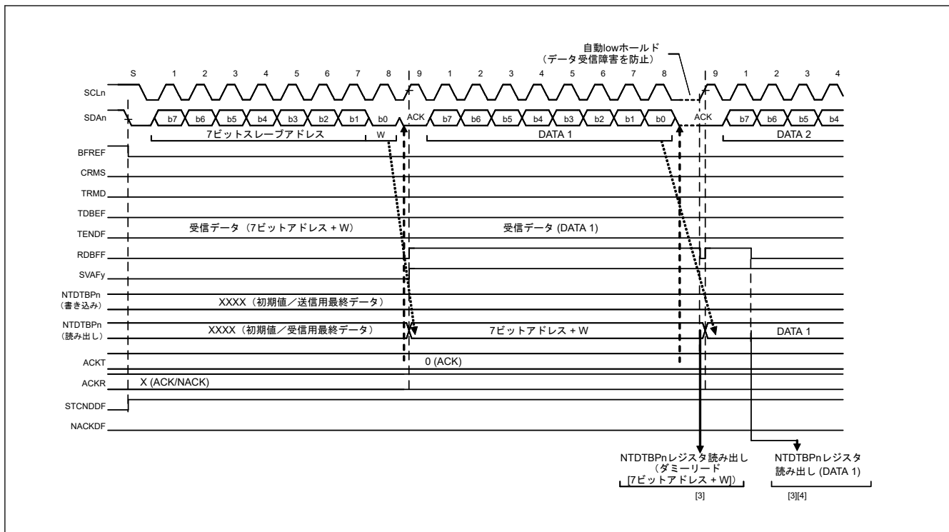
図 27.8 スレーブ受信の動作タイミング (1) (7 ビットアドレスフォーマットで ACKTWE = 0 の場合)
