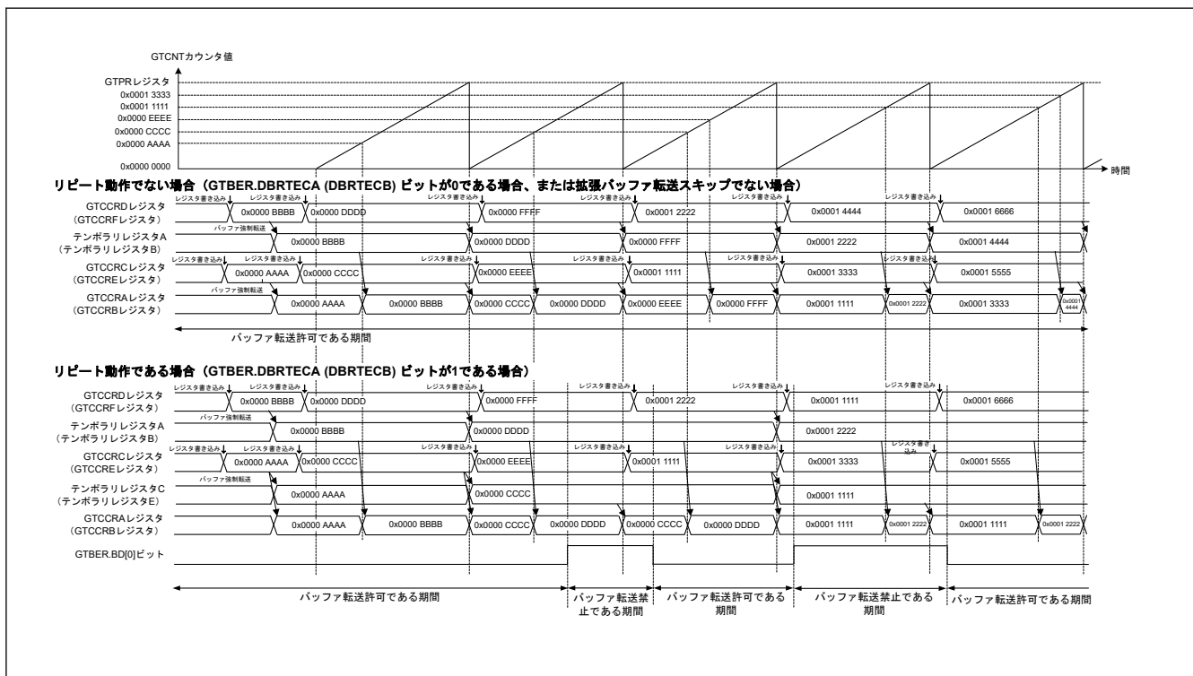
図 21.168 GTCCR バッファ転送禁止時のリピートダブルバッファ動作例 (のこぎり波ワンショットパルスモード、GTBER.BD[0]ビット更新の場合)
