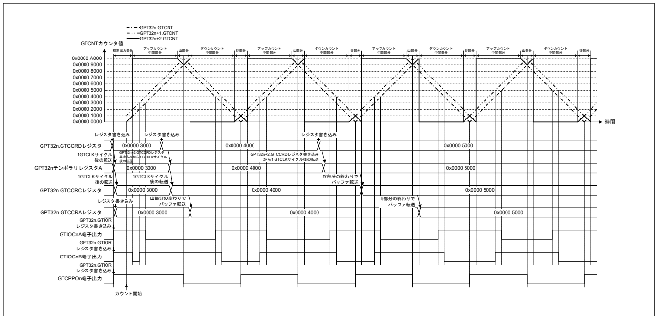
図 21.48 相補 PWM モード 1 動作例 (初期出力時 : GTIOCnA 端子 = High/GTIOCnB 端子 = High、アップカウントの GTCCRA レジスタコンペアマッチ時 : GTIOCnA 端子 = Low/GTIOCnB 端子 = High、ダウンカウントの GTCCRA レジスタコンペアマッチ時 : GTIOCnA 端子 = High/GTIOCnB 端子 = Low、デッドタイム値 : 0x0000 1000、GTCCRD レジスタを中間部分で更新) (n = 4、7)
