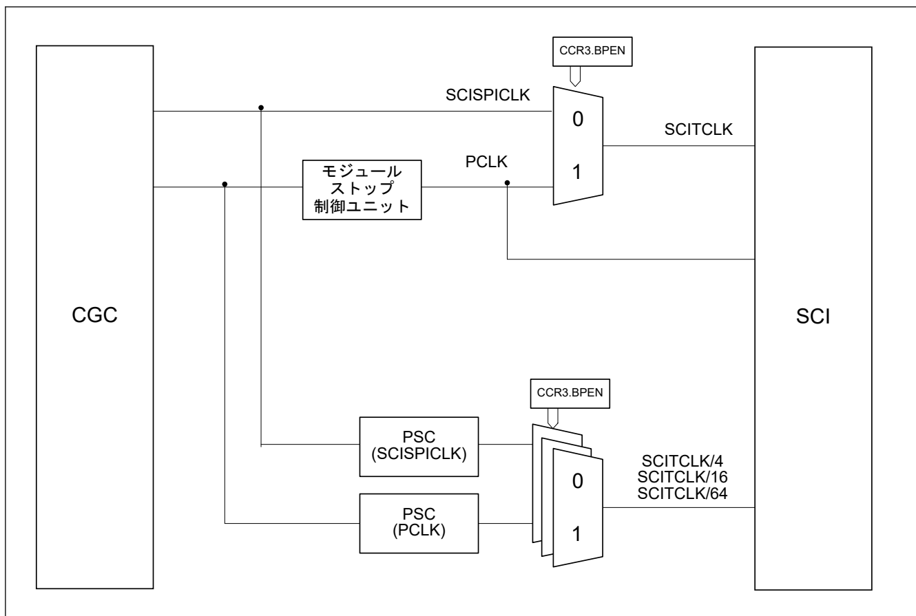
図 26.2 クロックソースセレクトアのブロック図
