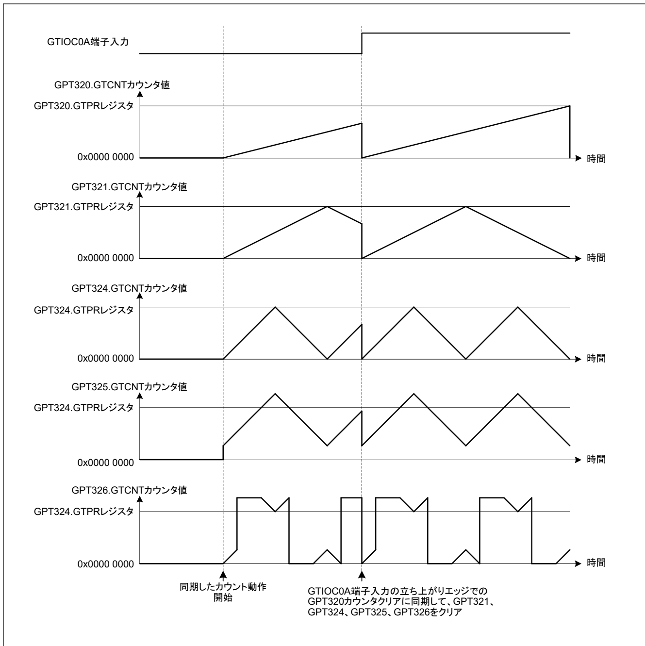
図 21.110 チャネル間連携による同期クリア動作例 (GTIOCnA/GTIOCnB 端子によるクリア) (GPT320 がのこぎり波、GTIOC0A の立ち上がりエッジでカウンタクリア、GPT321 が三角波、GPT324、GPT325、GPT326 が相補 PWM モード、GPT320、GPT321、GPT324、GPT325、GPT326 は同じ同期セット / クリアグループ)
