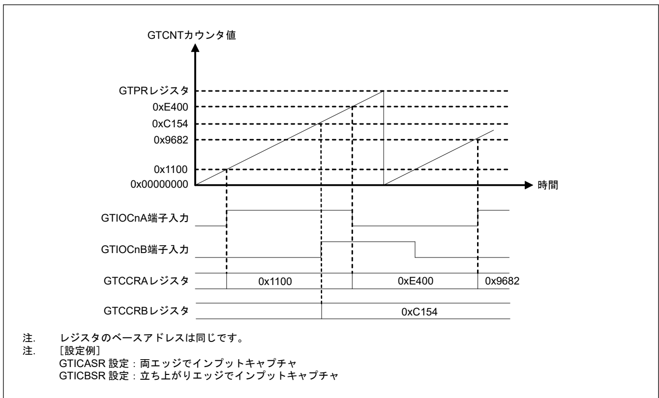
図 21.14 インพุットキャプチャ動作例
