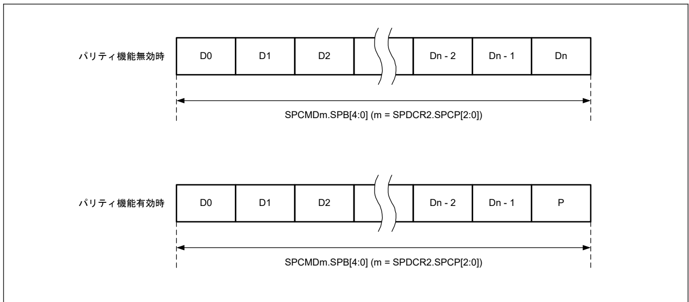
図 30.14 パリティ機能無効時と有効時のデータフォーマット
