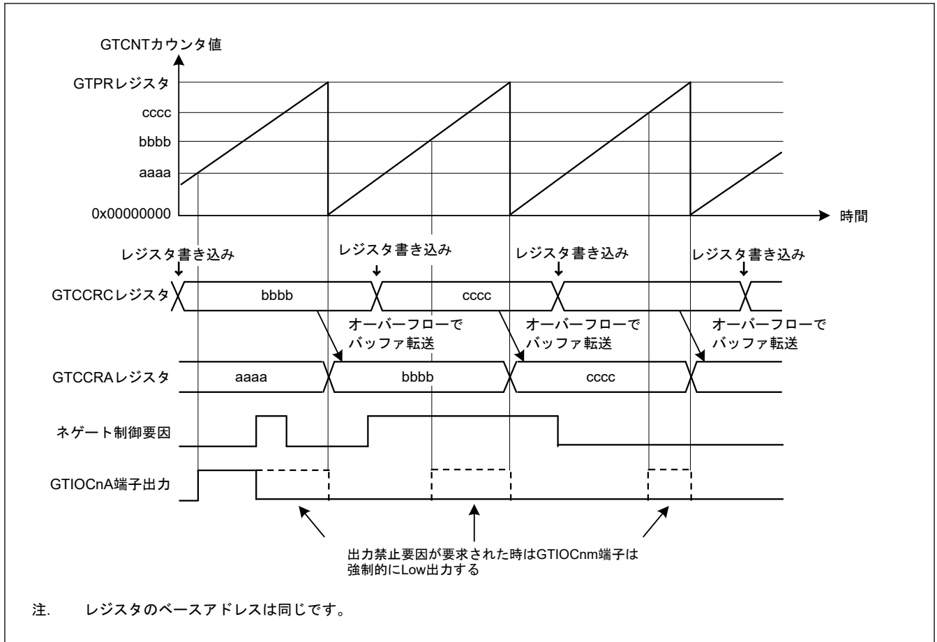
図 21.171 GTIOcnm 端子出力禁止制御動作例 (のこぎり波でアップカウント、バッファ動作、アクティブレベル 1、GTCCRA レジスタのコンペアマッチで High 出力、周期の終わりで Low 出力、出力禁止で Low 出力の場合) (n = 0~9, m = A, B)
