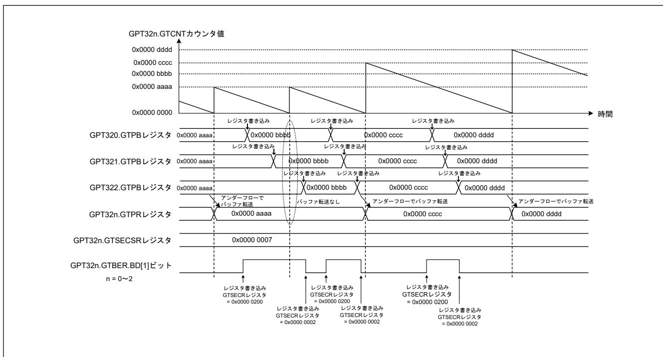
図 21.166 バッファ動作禁止の複数チャンネルの動作例 (のこぎり波、シングルバッファ動作)
