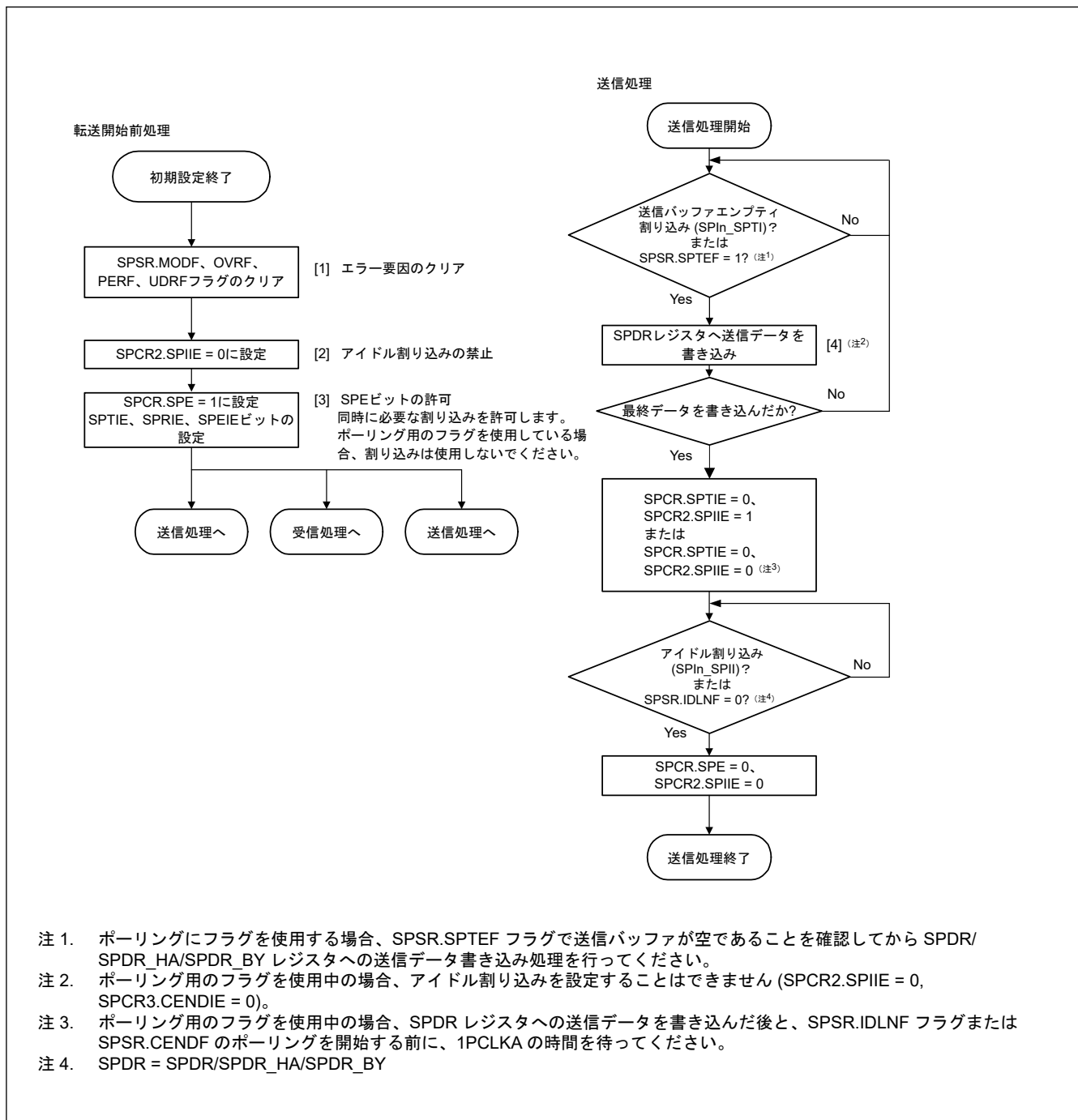
図 29.49 マスタモードでの送信フロー
