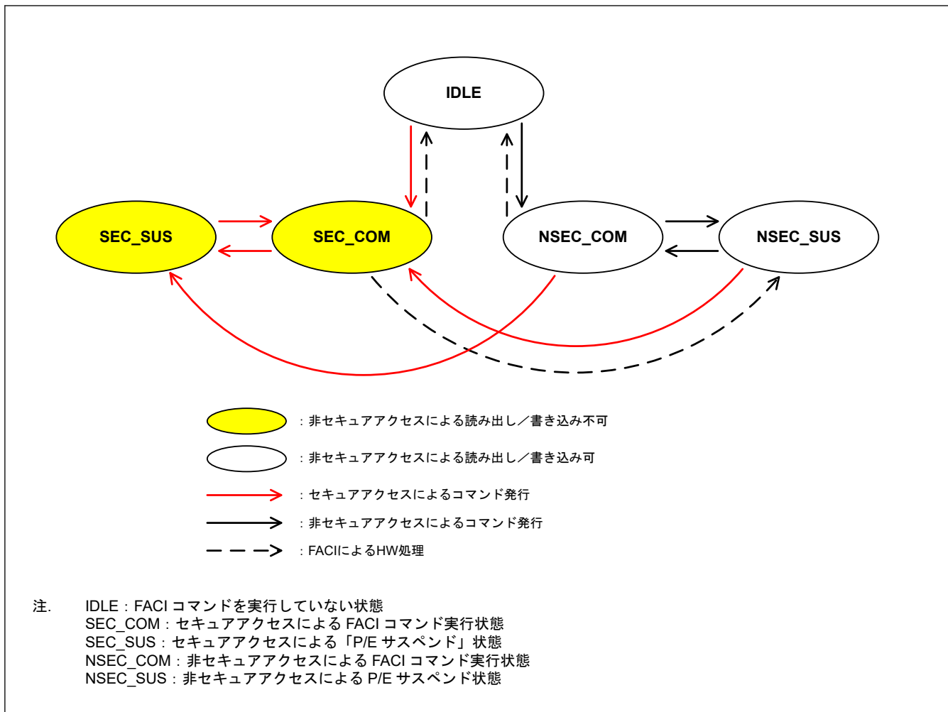
図 39.33 FACL コマンド動作中の保護状態
