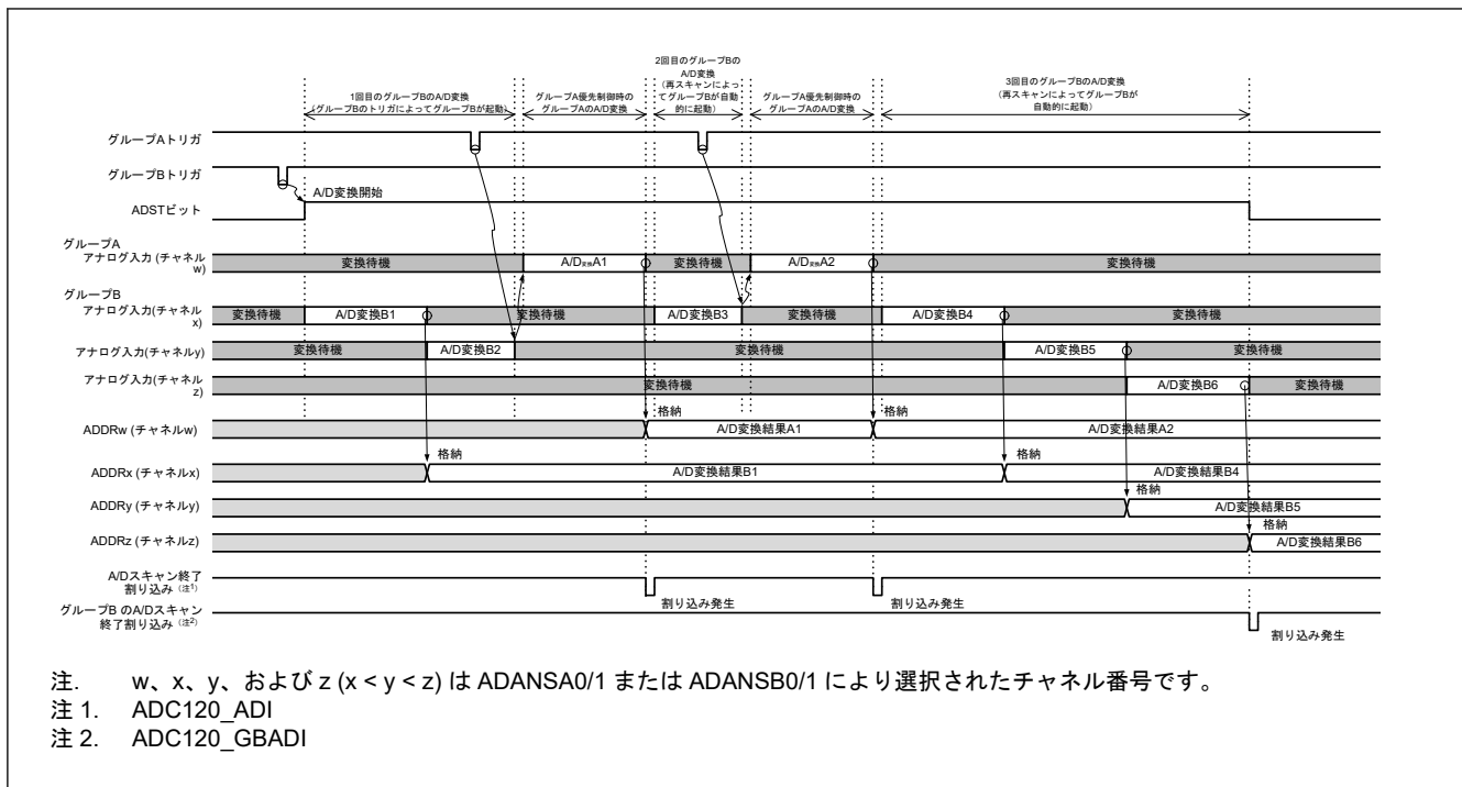
図 33.27 グループ優先動作例 1-2：グループ B 再スキャン中のグループ A トリガ入力、再スキャンあり (ADGSPCR.GBRSCN = 1、ADGSPCR.GBRP = 0、および ADGSPCR.LGRRS = 0 の場合)
