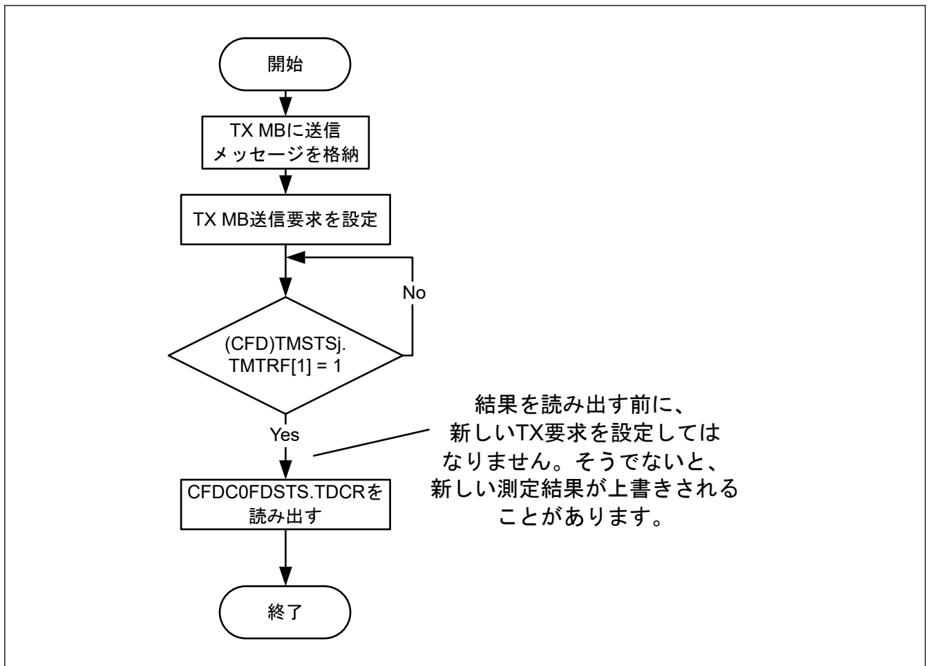
図 27.22 TDC 結果読み出しフロー
