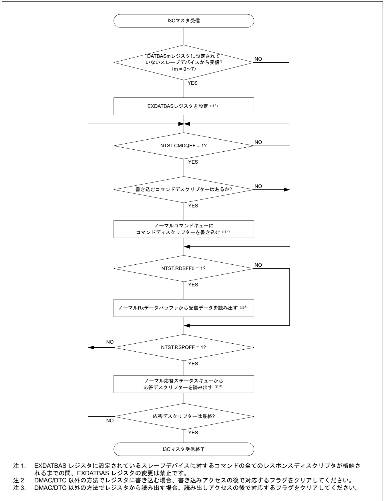
図 26.120 I3C マスタ受信のフローチャート例 (通常 FIFO バッファ転送)
