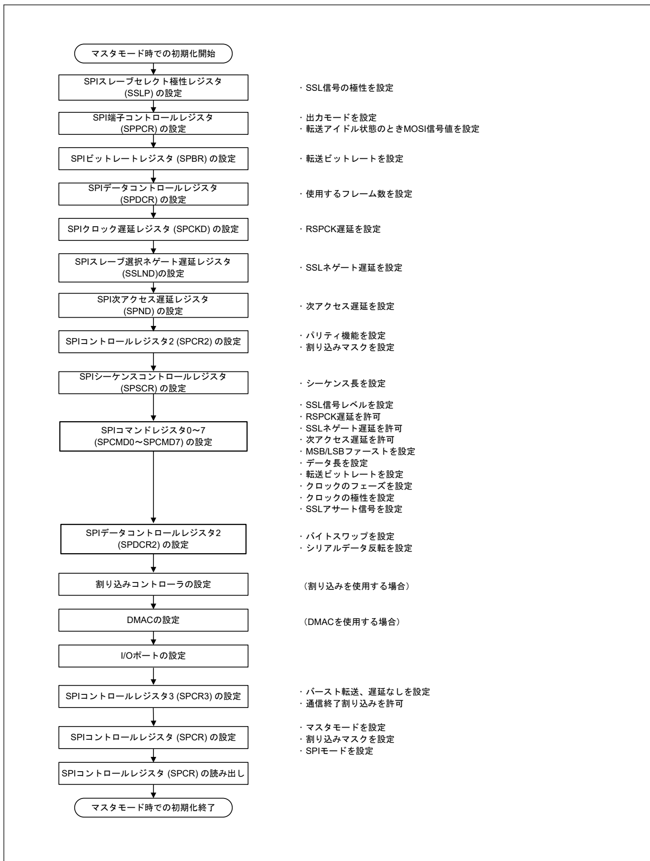
図 29.48 マスタモード時の SPI 動作の初期化フロー例
