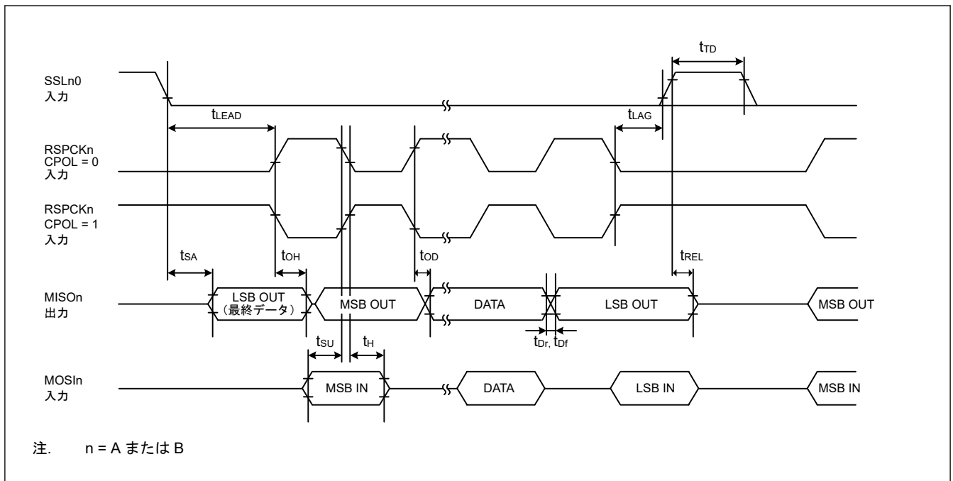
図 42.40 CPHA = 1 の場合におけるスレーブの SPI タイミング
