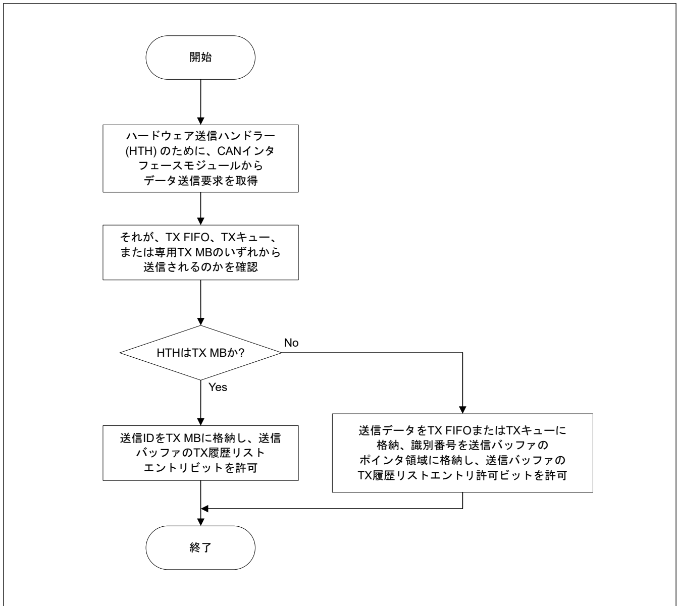
図 27.50 TX 履歴リストの準備手順
