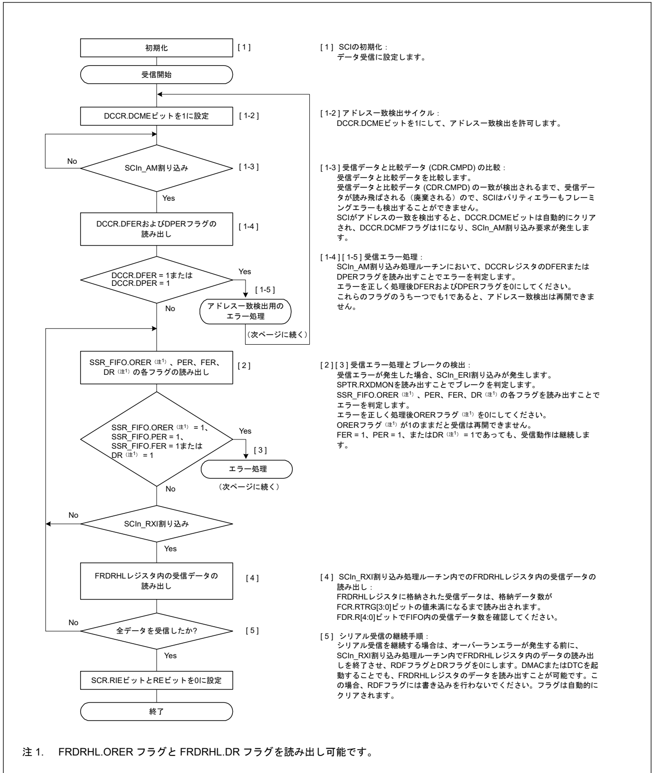
図 25.25 調歩同期式モードにおけるシリアル受信のフローチャート例 (FIFO 選択、アドレス一致検出有効時) (1)
