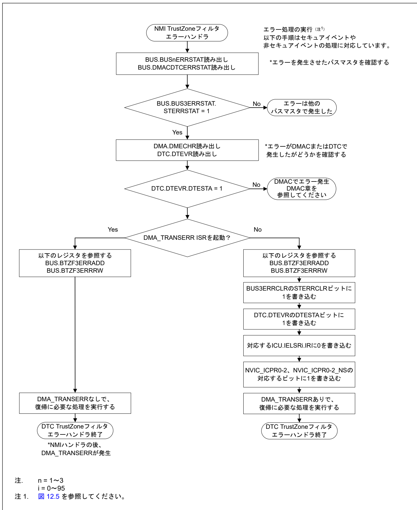
図 16.15 スレープ TrustZone フィルタエラーの NMI ハンドラにおける処理
