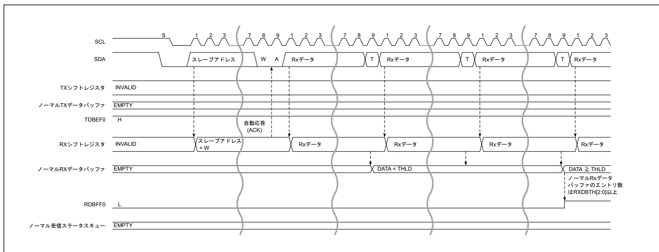
図 26.35 SDR データ書き込み転送タイミング (1/2)
