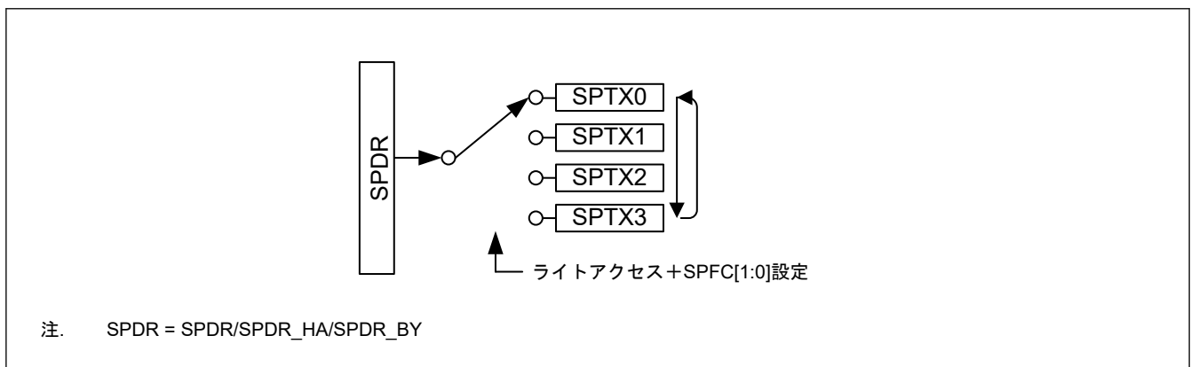
図 29.3 書き込み時の SPDR/SPDR_HA/SPDR_BY レジスタの構成図
