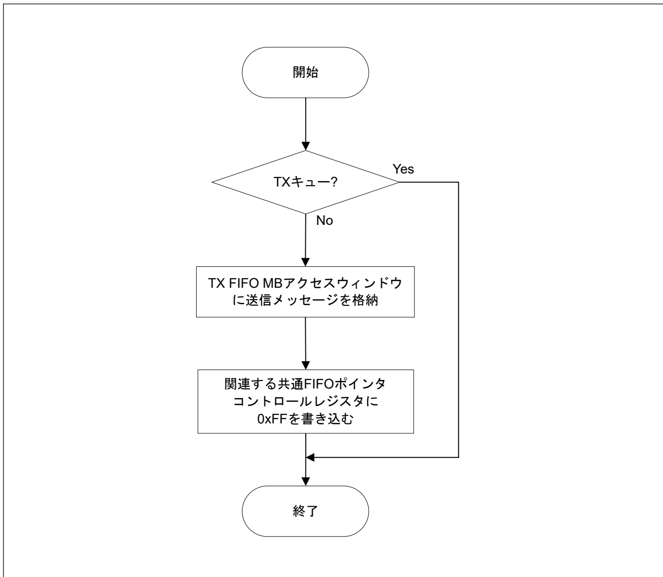
図 27.46 TX FIFO の送信要求手順
