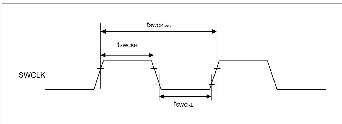
図 42.62 SWD SWCLK タイミング
