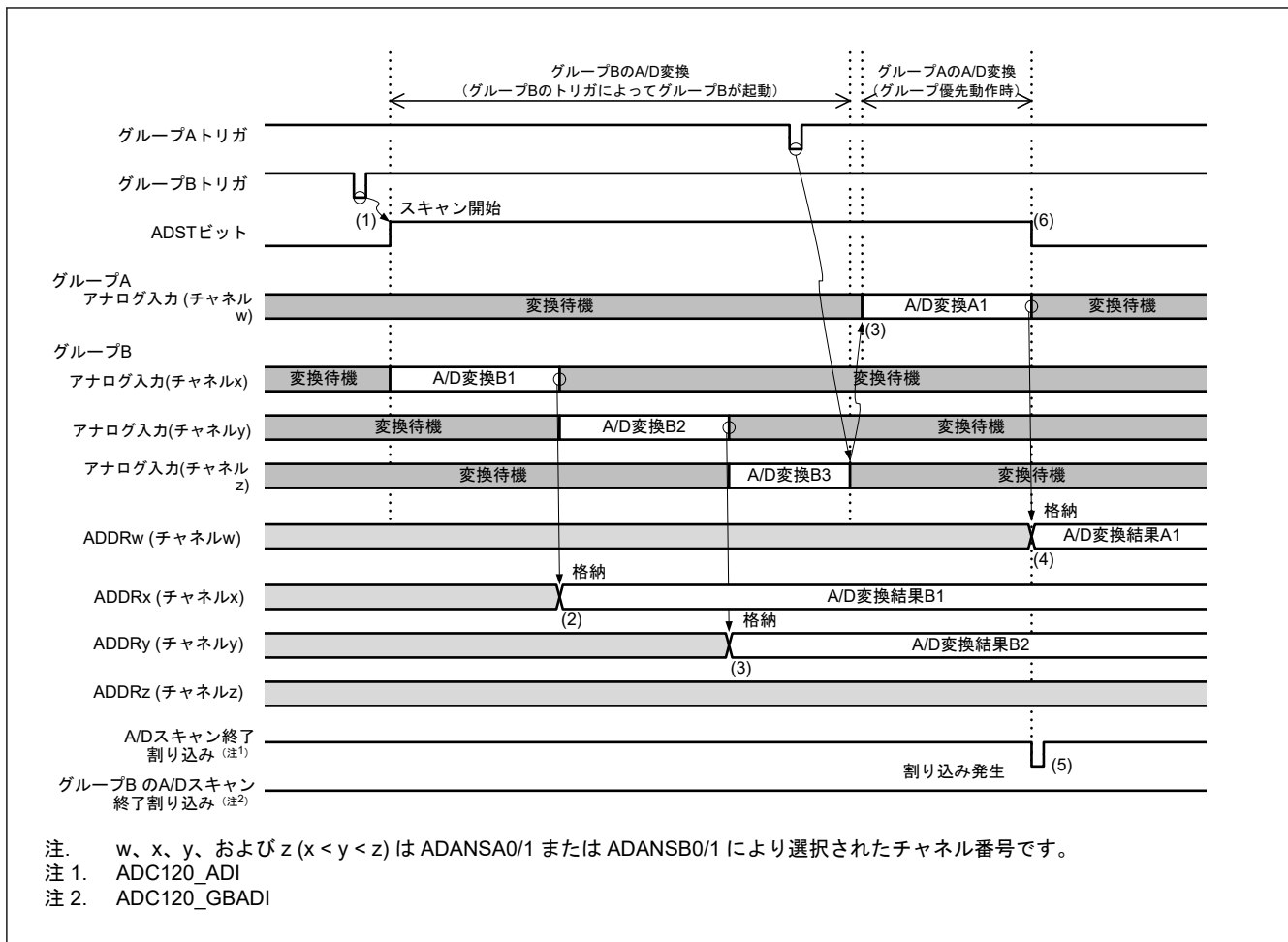
図 33.29 グループ優先動作例 1-4：グループ B スキャン中のグループ A トリガ入力、再スキャンなし (ADGSPCR.GBRSCN = 0、ADGSPCR.GBRP = 0、および ADGSPCR.LGRRS = 0 の場合)
