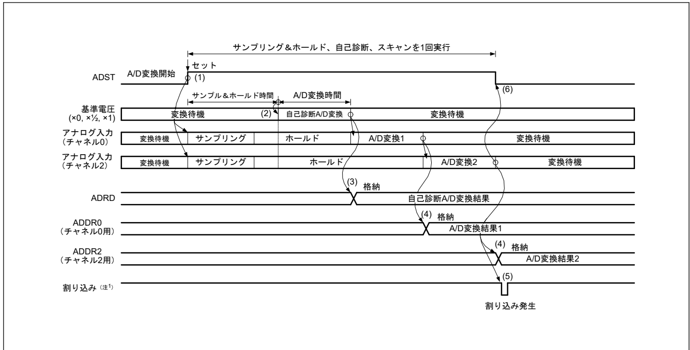
図 33.11 シングルスキャンモードの動作例（チャンネル専用サンプル&ホールド回路を使用し、自己診断で AN000 と AN002 を選択し、連続サンプリングを無効にした場合）
