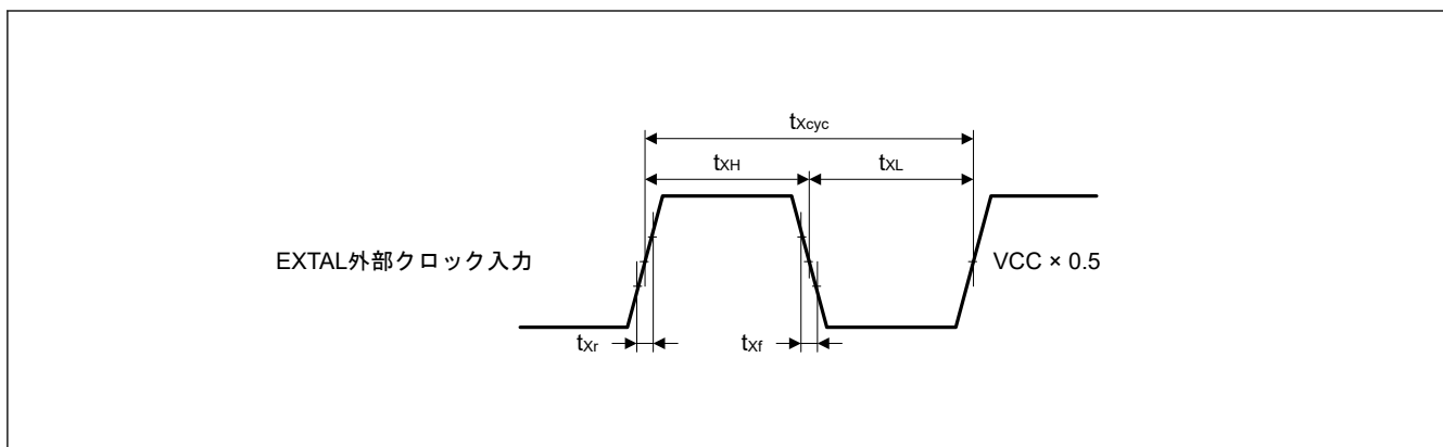
図 42.7 EXTERNAL 外部クロック入力タイミング
