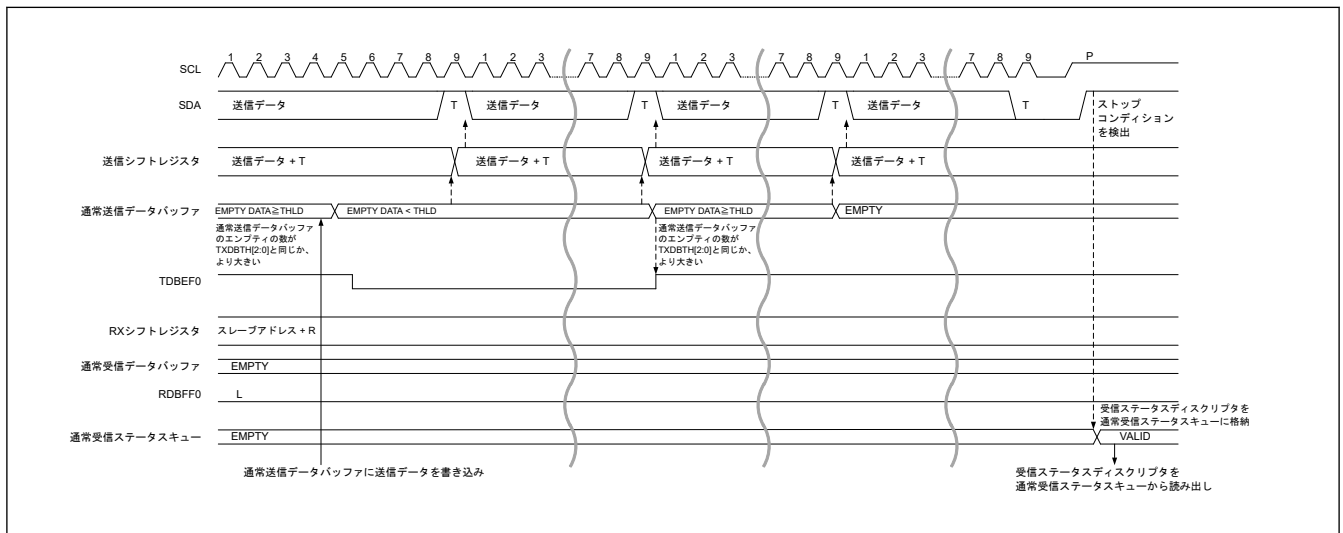
図 26.40 SDR データ読み出し転送タイミング (2/2)
