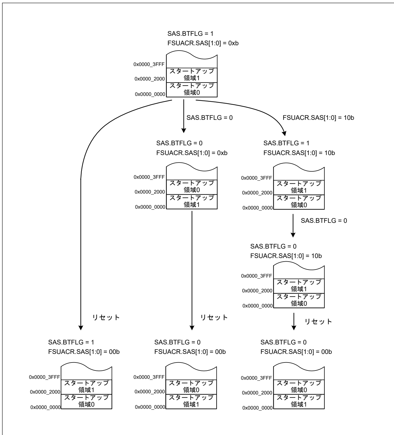
図 39.26 スタートアッププログラムプロテクション設定の遷移例 1
