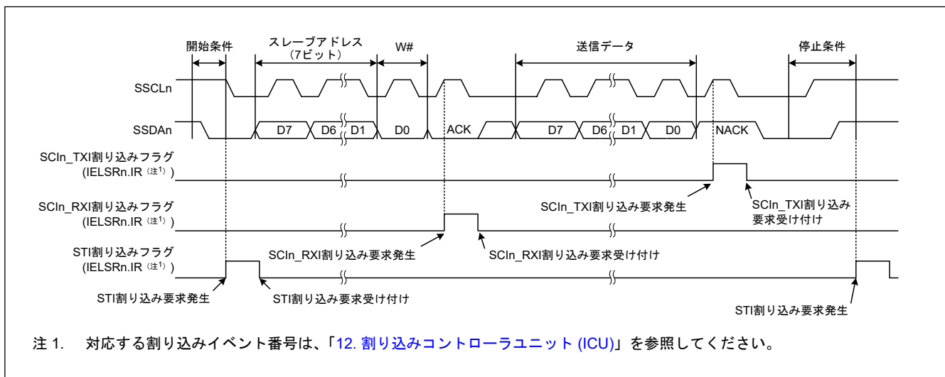
図 25.91 簡易 IIC モードにおけるマスタ送信の動作例 2 (7 ビットスレーブアドレス、ACK 割り込み、NACK 割り込み使用時)
