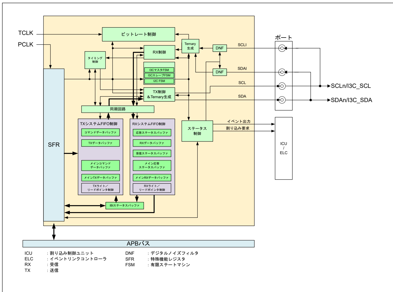
図 26.1 I3C ブロック図
