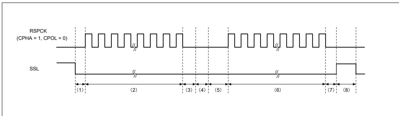
図 29.46 SSLKP ビット(BFDS = 0) を利用したバースト転送の動作例
