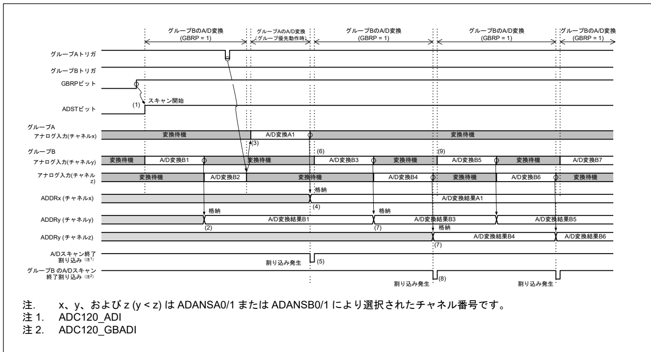
図 33.30 グループ優先動作例 1-5: グループ B のシングルスキャン連続動作 (ADGSPCR.GBRP = 1、ADGSPCR.LGRRS = 0 の場合)
