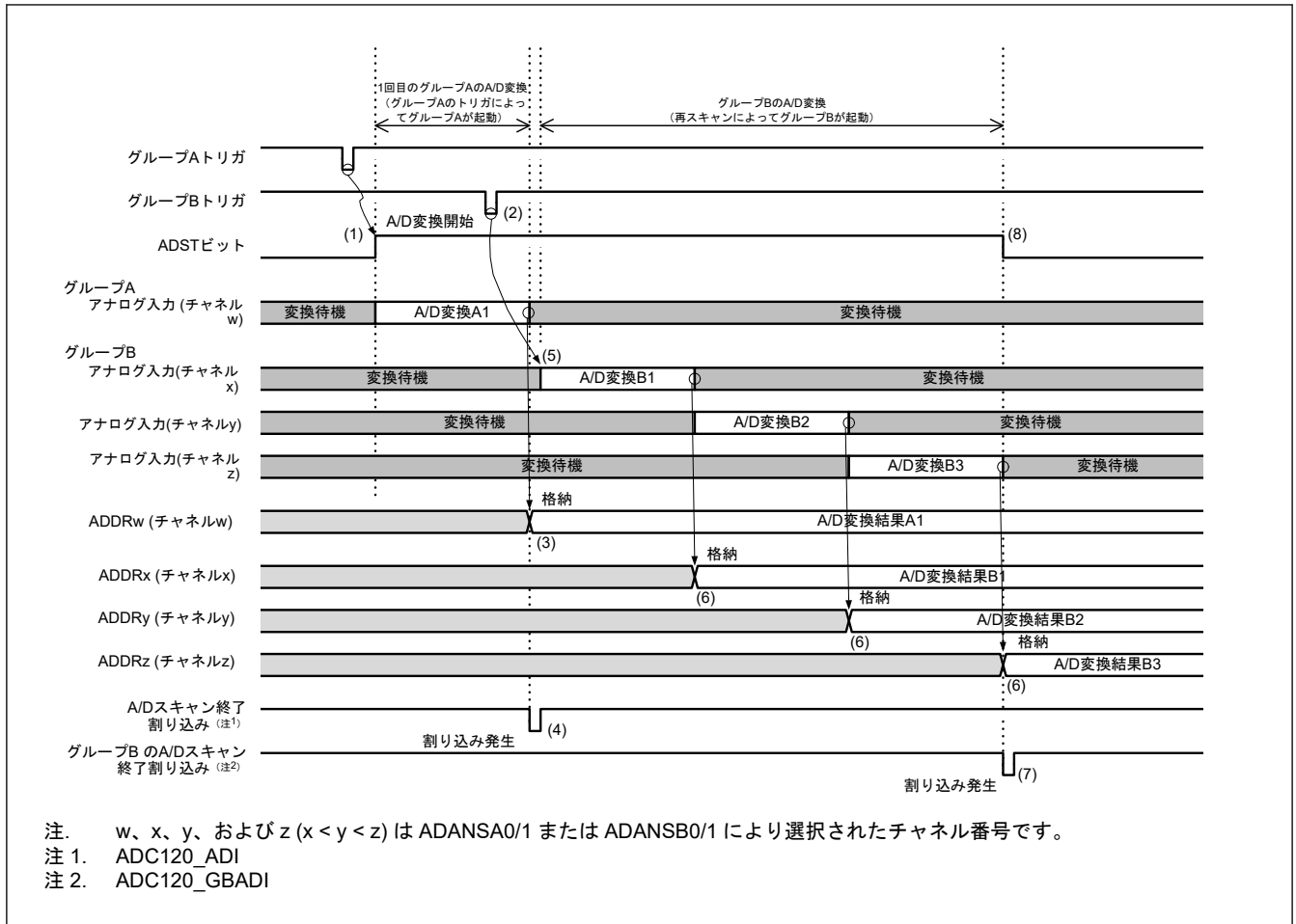
図 33.28 グループ優先動作例 1-3：グループ A スキャン中のグループ B トリガ入力、再スキャンあり (ADGSPCR.GBRSCN = 1、ADGSPCR.GBRP = 0、および ADGSPCR.LGRRS = 0 の場合)
