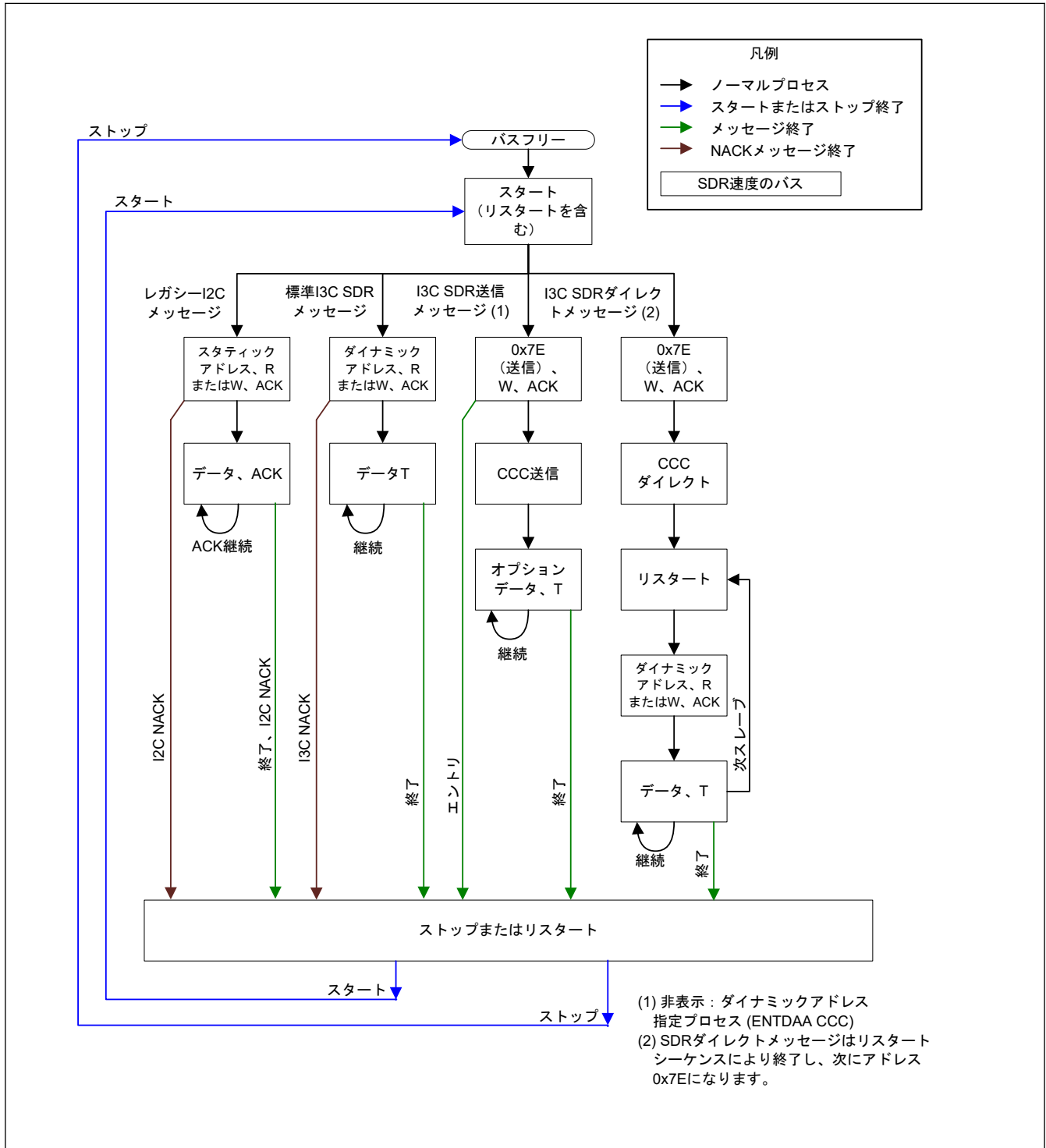
図 26.115 I3C 通信フロー
