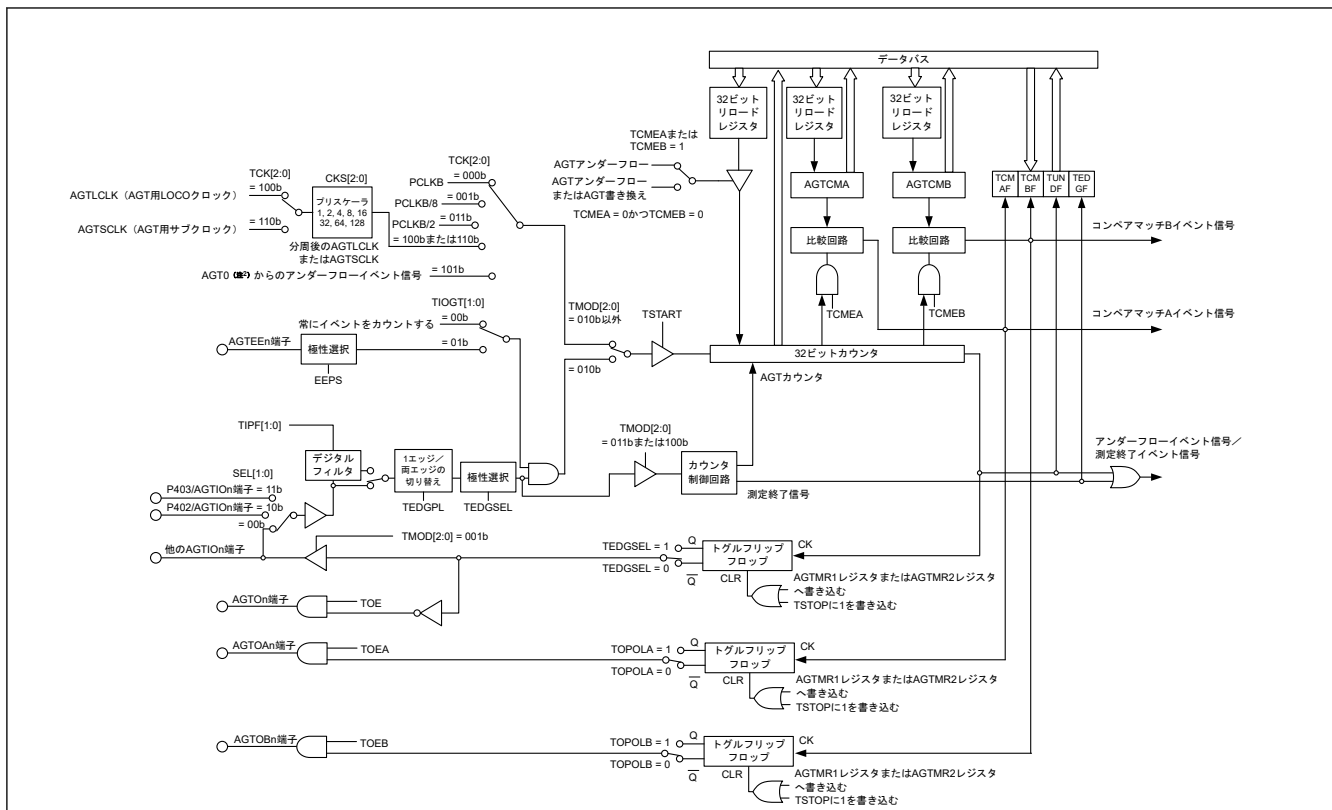
図 21.1 AGT のブロック図
