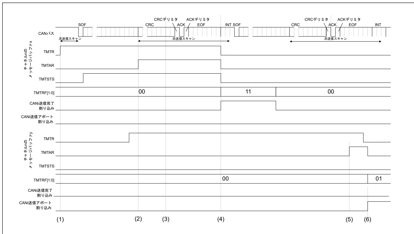
図 27.45 送信アボートの要求およびフラグビットのタイミング
