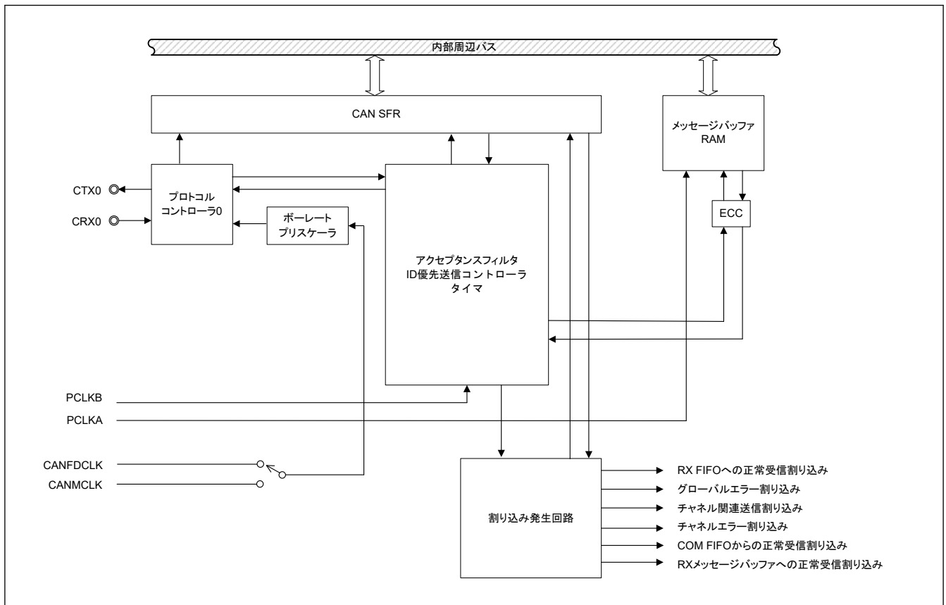
図 27.1 CANFD モジュールの概要
