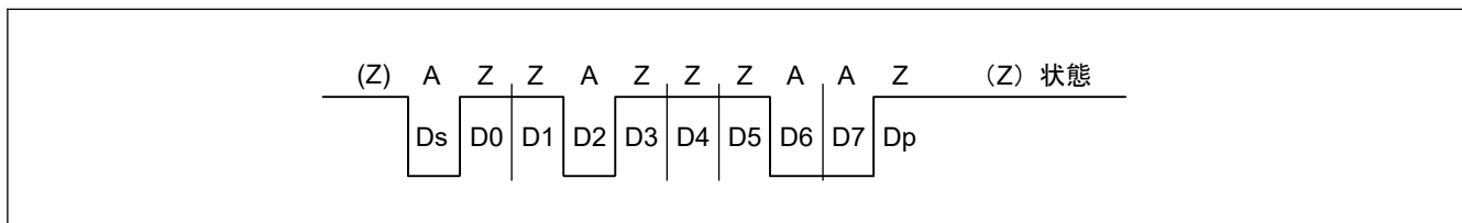
図 25.76 ダイレクトコンベンション (SCMR.SDIR ビット = 0、SCMR.SINV ビット = 0、SMR_SMCI.PM ビット = 0)
