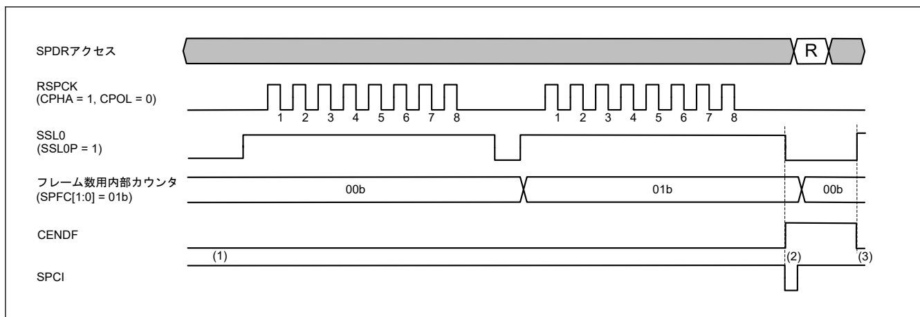
図 29.33 通信終了割り込み動作例 (SPI 動作時の受信のみスレーブモード)
