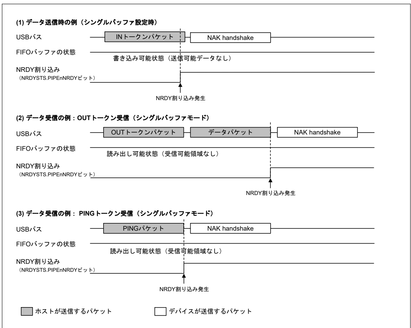
図 24.9 NRDY 割り込み発生タイミング
