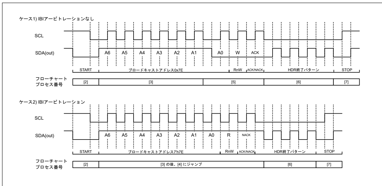
図 26.98 I3C マスタの I3C エスカレーション処理タイミングチャート
