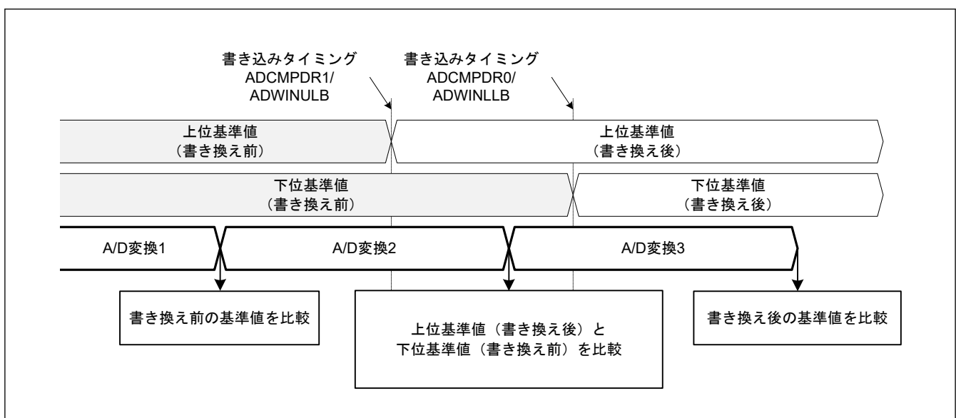
図 33.4 書き換え前後の上側基準値と下側基準値の比較
