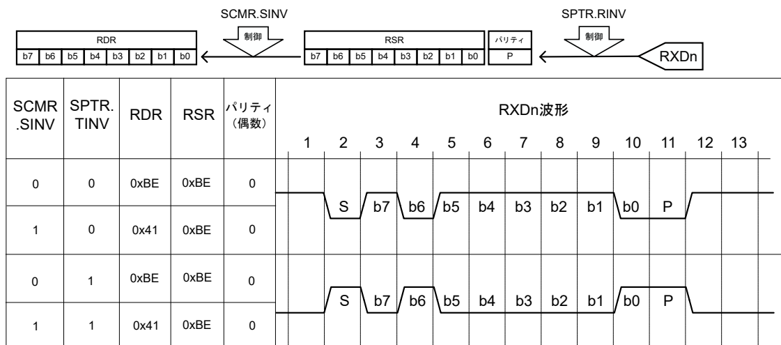
図 25.2 受信/送信データ制御の例
