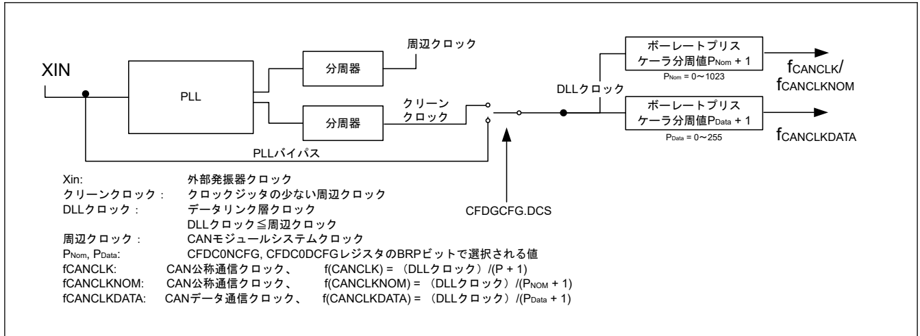
図 27.16 CAN チャンネルの通信クロックを生成する回路のブロック図
