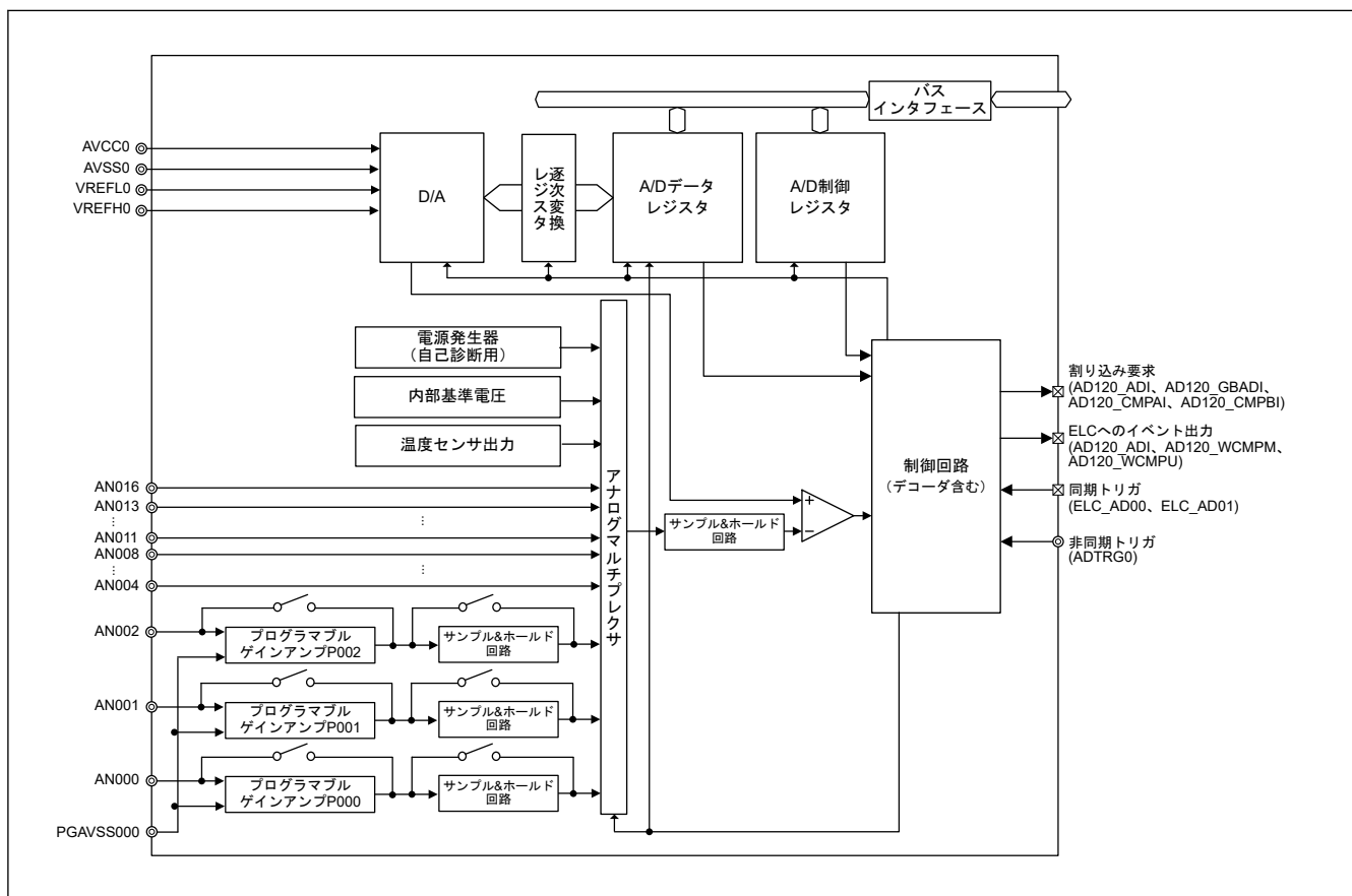
図 33.1 ADC12 のブロック図
