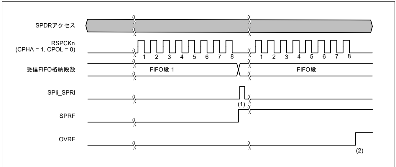
図 33.32 SPCR.TXMD[1:0] = 10b の場合の動作例
