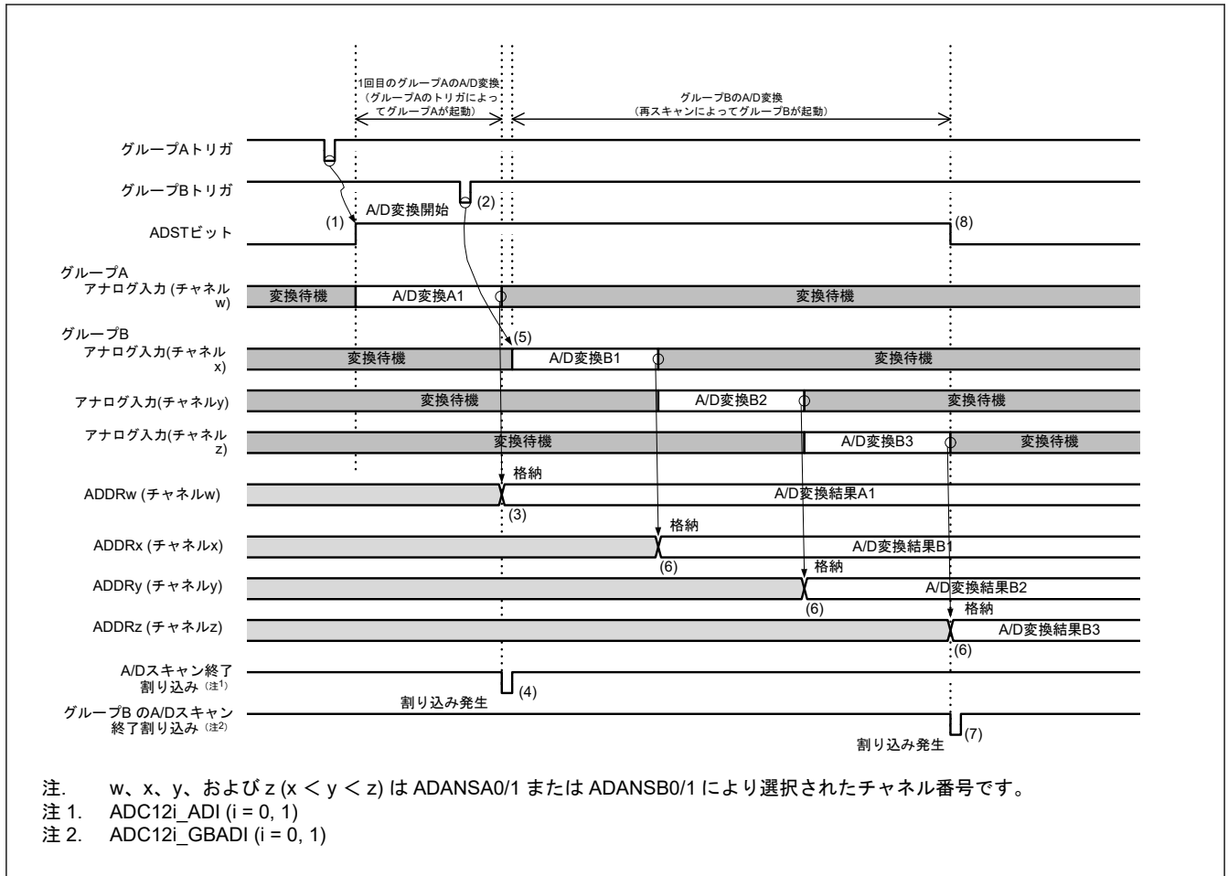
図 39.29 グループ優先動作の例 1-3 : グループ A スキャン中のグループ B トリガ入力、再スキャンあり (ADGSPCR.GBRSCN = 1、ADGSPCR.GBRP = 0、および ADGSPCR.LGRRS = 0 の場合)
