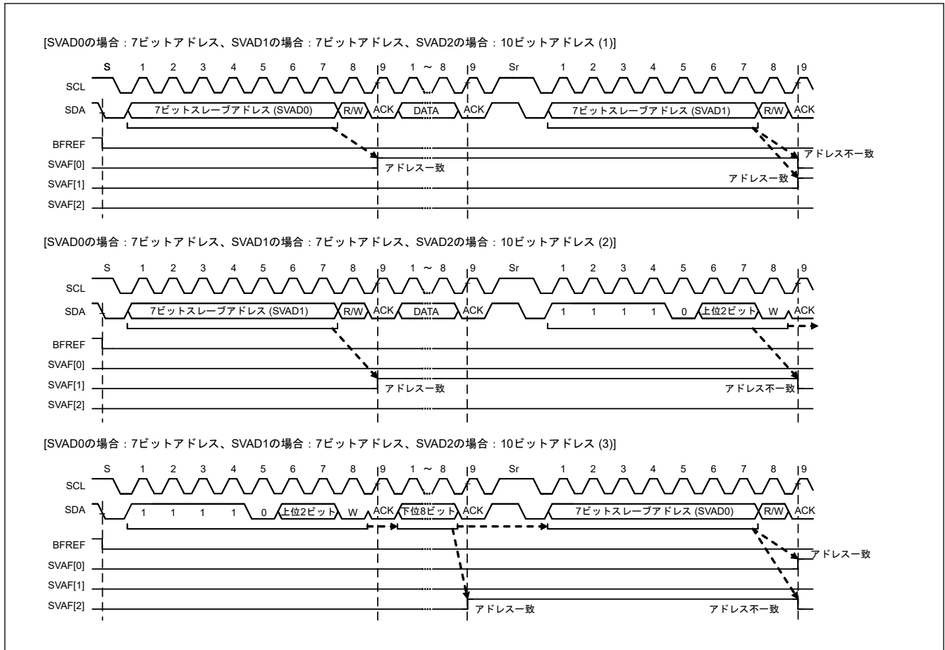
図 30.84 SVAy フラグが 1 または 0 になるタイミング (7 ビット/10 ビットアドレスフォーマット混在時)
