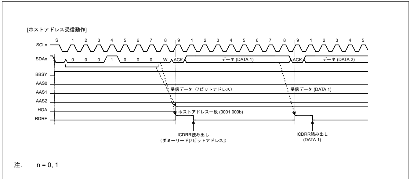
図 29.29 ホストアドレス受信時に HOA フラグが 1 になるタイミング
