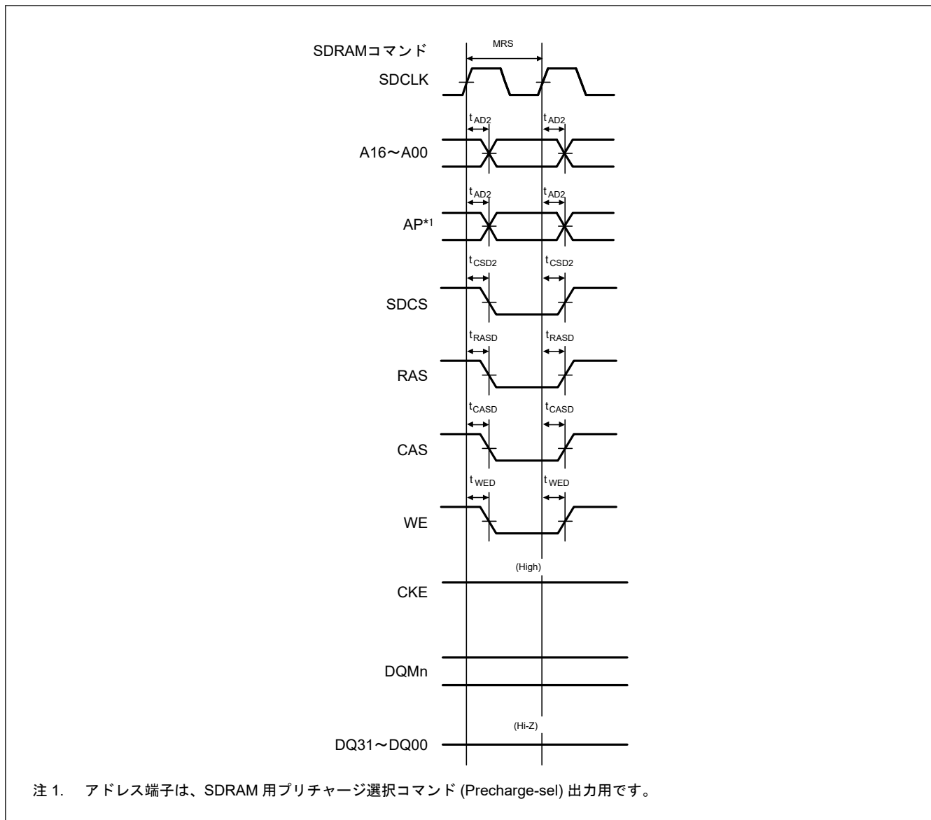
図 48.40 SDRAM モードレジスタの設定のタイミング
