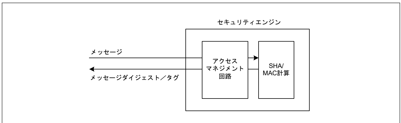
図 38.4 ハッシュ生成部の概念図
