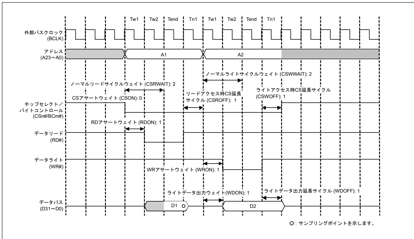
図 13.5 ノーマルアクセスの動作例（リード/ライト）(n = 0~7, m = 0~3)
