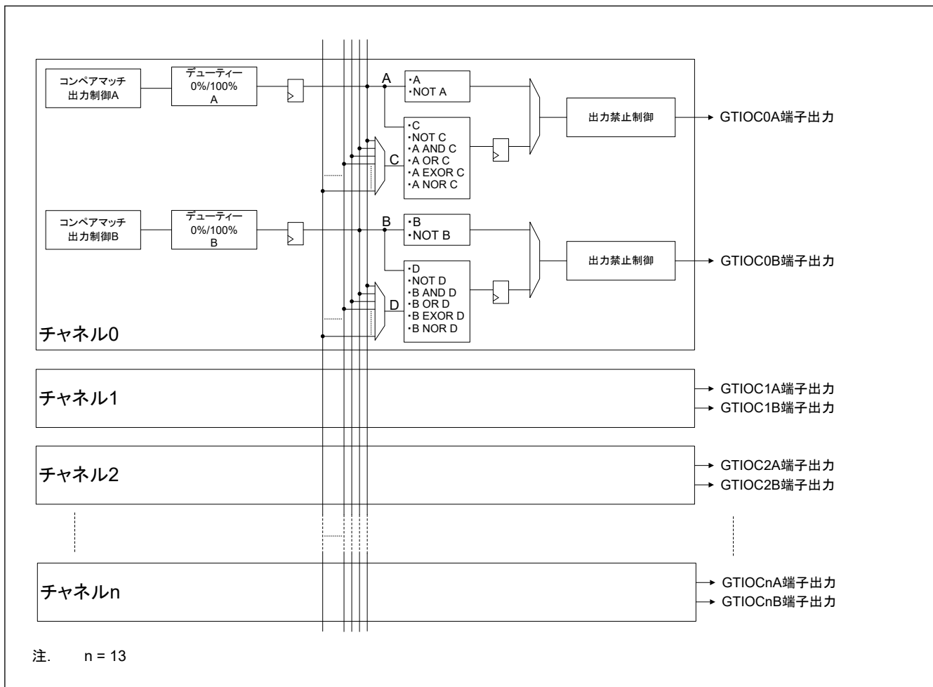
図 20.68 チャネル間論理演算のブロック図
