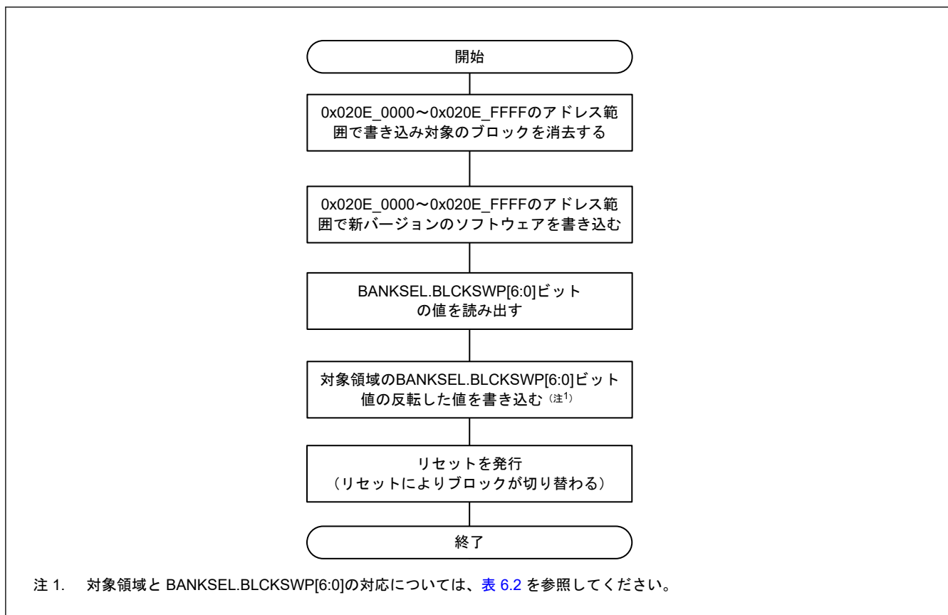
図 46.36 セキュアエイリアスのブロックスワップ選択フロー例 (2 MB のコードフラッシュメモリを持つ製品の場合)
