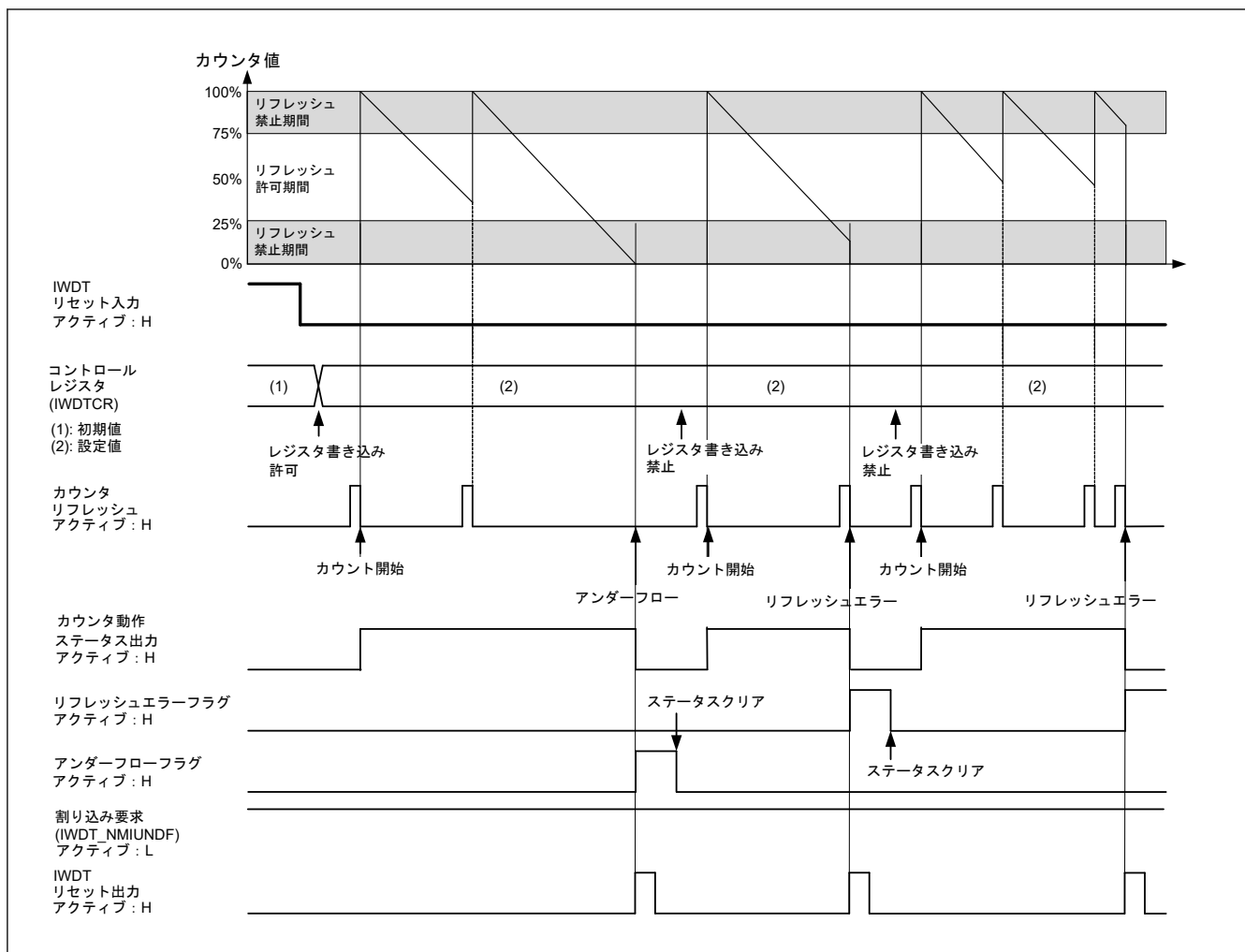
図 24.3 レジスタスタートモードでの動作例
