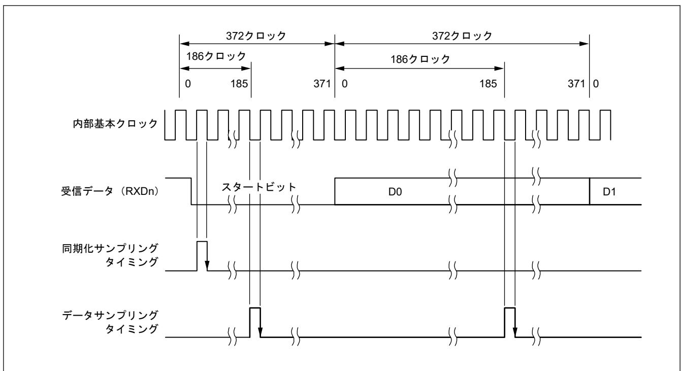
図 28.78 スマートカードインタフェースモードにおける受信データのサンプリングタイミング（ビットレートの 372 倍のクロック周波数の場合）
