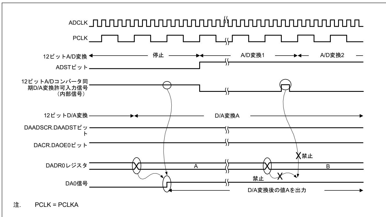
図 40.4 DAC12 が次からの同期 D/A 変換許可入力信号を取り込めない場合の例：ADC12 (ユニット 1)
