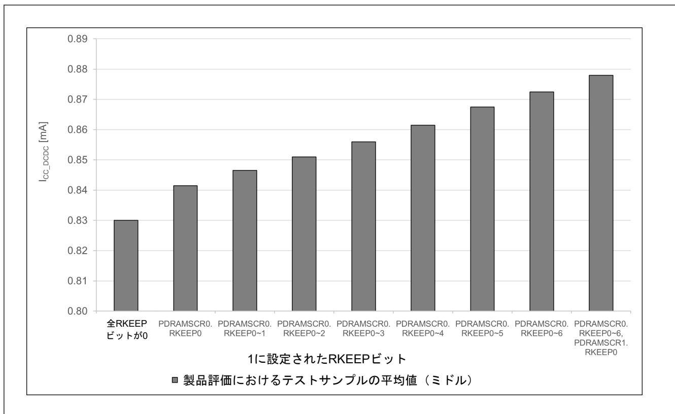
図 48.8 1 SRAM ステートあたりのソフトウェアスタンバイ電流 (参考データ)
