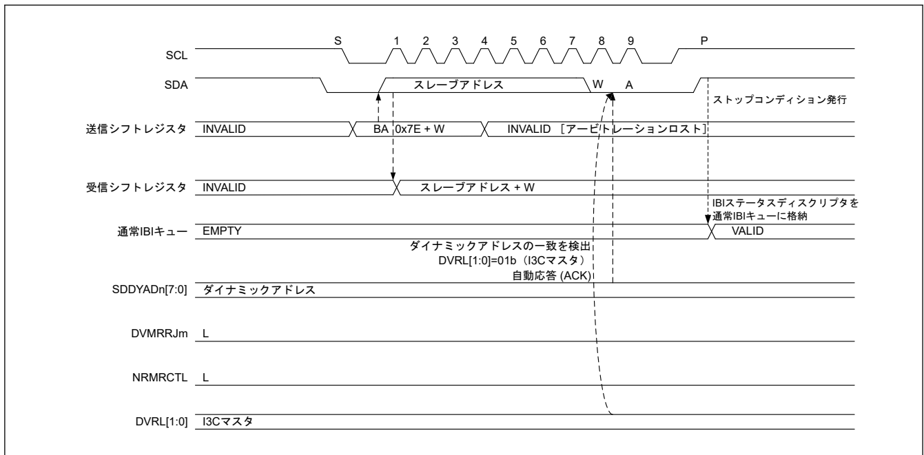
図 30.105 バス権要求 : ACK
