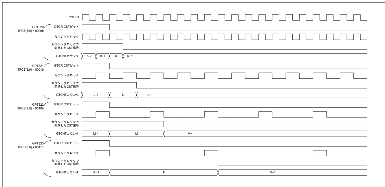
図 20.41 ソフトウェアによる同時ストップの動作例 (異なるカウント周期)
