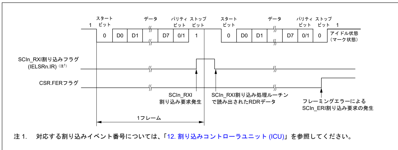
図 28.19 調歩同期式モードにおけるシリアル受信の動作例 (1) (RTS 機能を使用しない場合) (8 ビットデータ / パリティあり / 1 ストップビットの場合)
