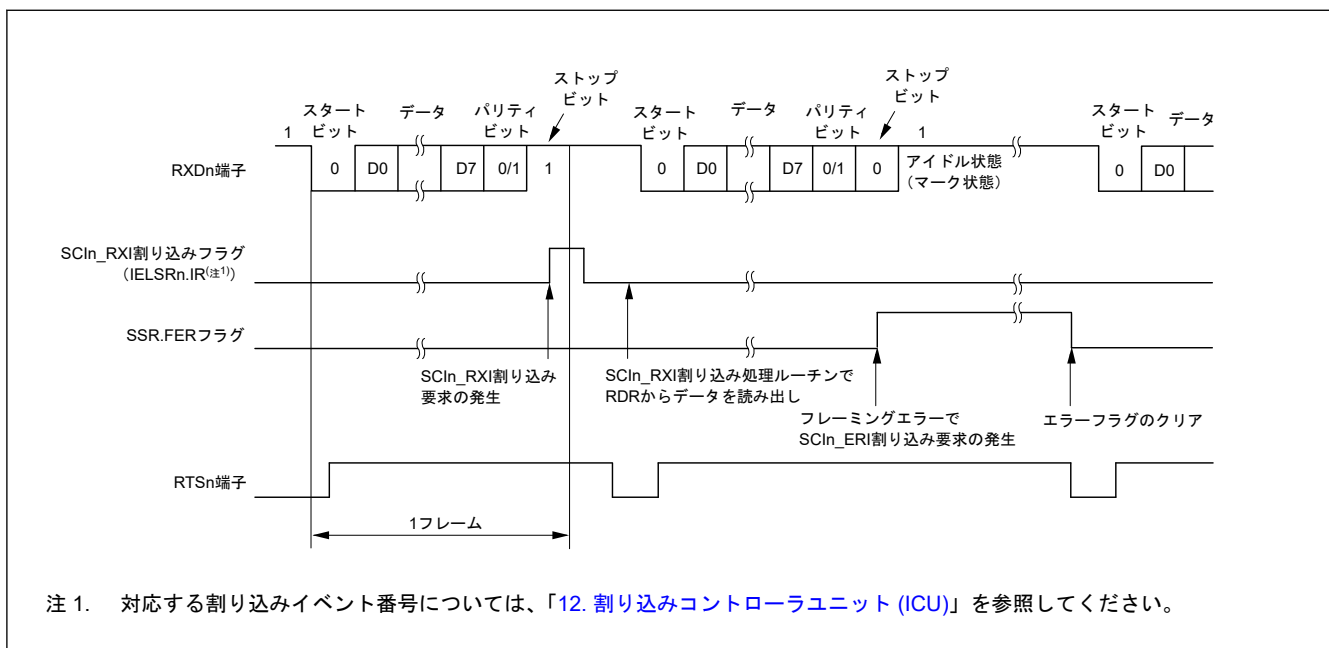
図 28.20 調歩同期式モードにおけるシリアル受信の動作例 (2) (RTS 機能を使用する場合) (8 ビットデータ / パリティあり / 1 ストップビットの場合)
