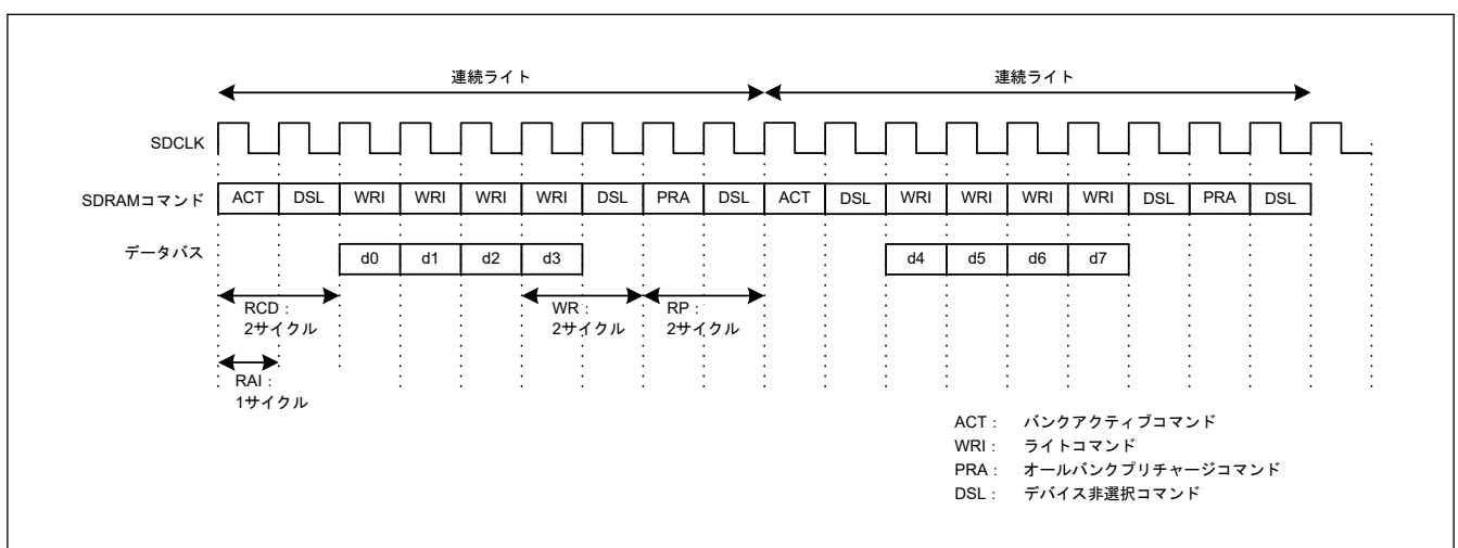
図 13.67 連続ライトタイミング例 (3)
