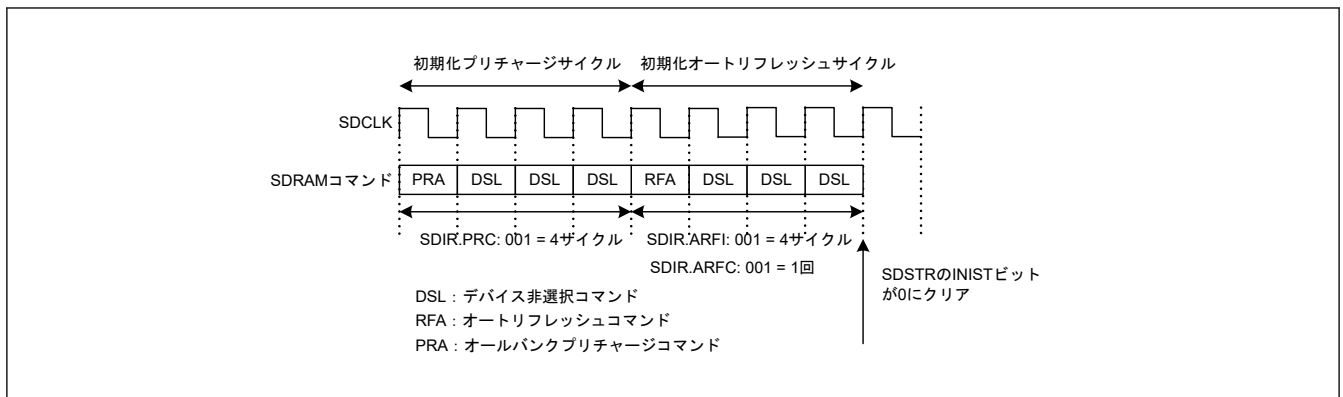
図 13.42 SDRAM 初期化シーケンスのタイミング例
