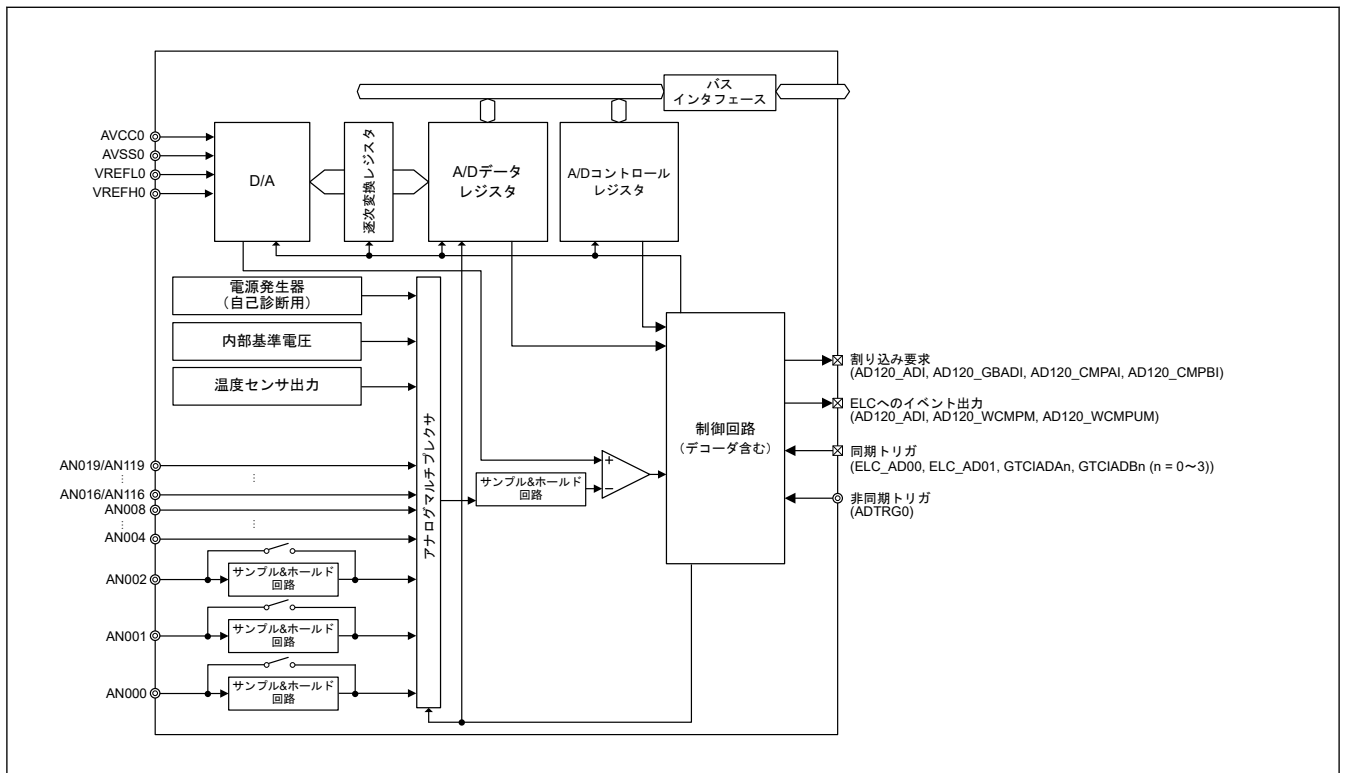
図 39.1 ADC12 ブロック図 (ユニット 0)
