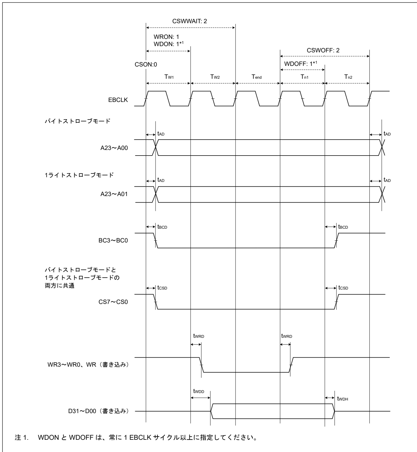
図 48.31 バスロック同期を使用したノーマルライトサイクルの外部バスタイミング
