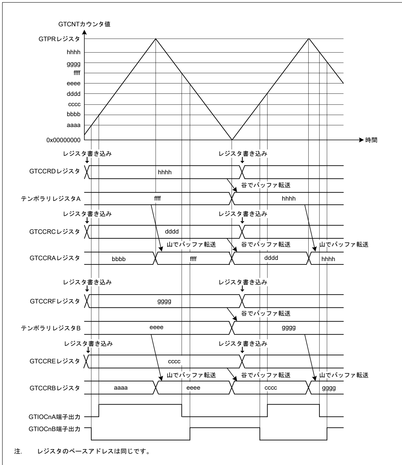
図 20.25 三角波 PWM モード 3 の動作例 (カウントスタート時に GTIOcNA 端子 = Low 出力/GTIOcNB 端子 = High 出力、GTCRA/GTCRB レジスタのコンペアマッチ時にトグル出力、周期の終わりで出力保持の場合)
