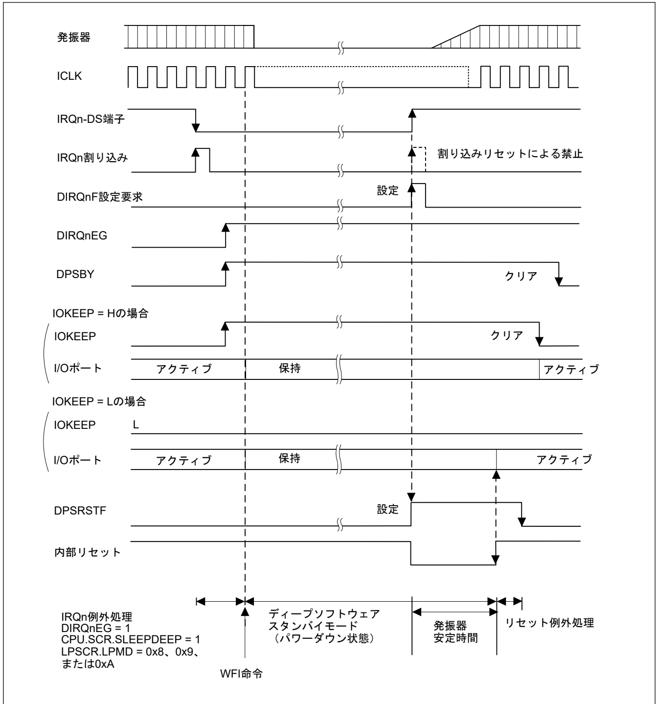
図 10.4 ディープソフトウェアスタンバイモードの応用例
