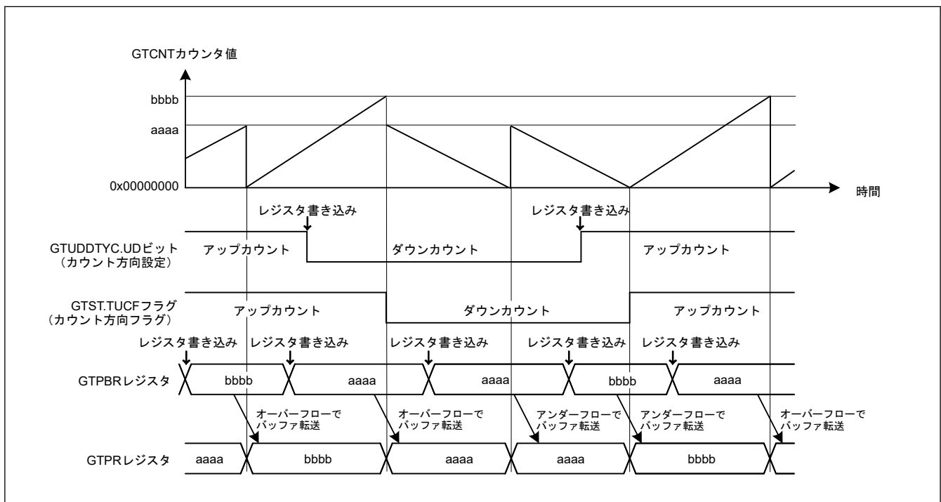
図 20.30 カウント方向切り替え機能の動作例（バッファ動作時）
