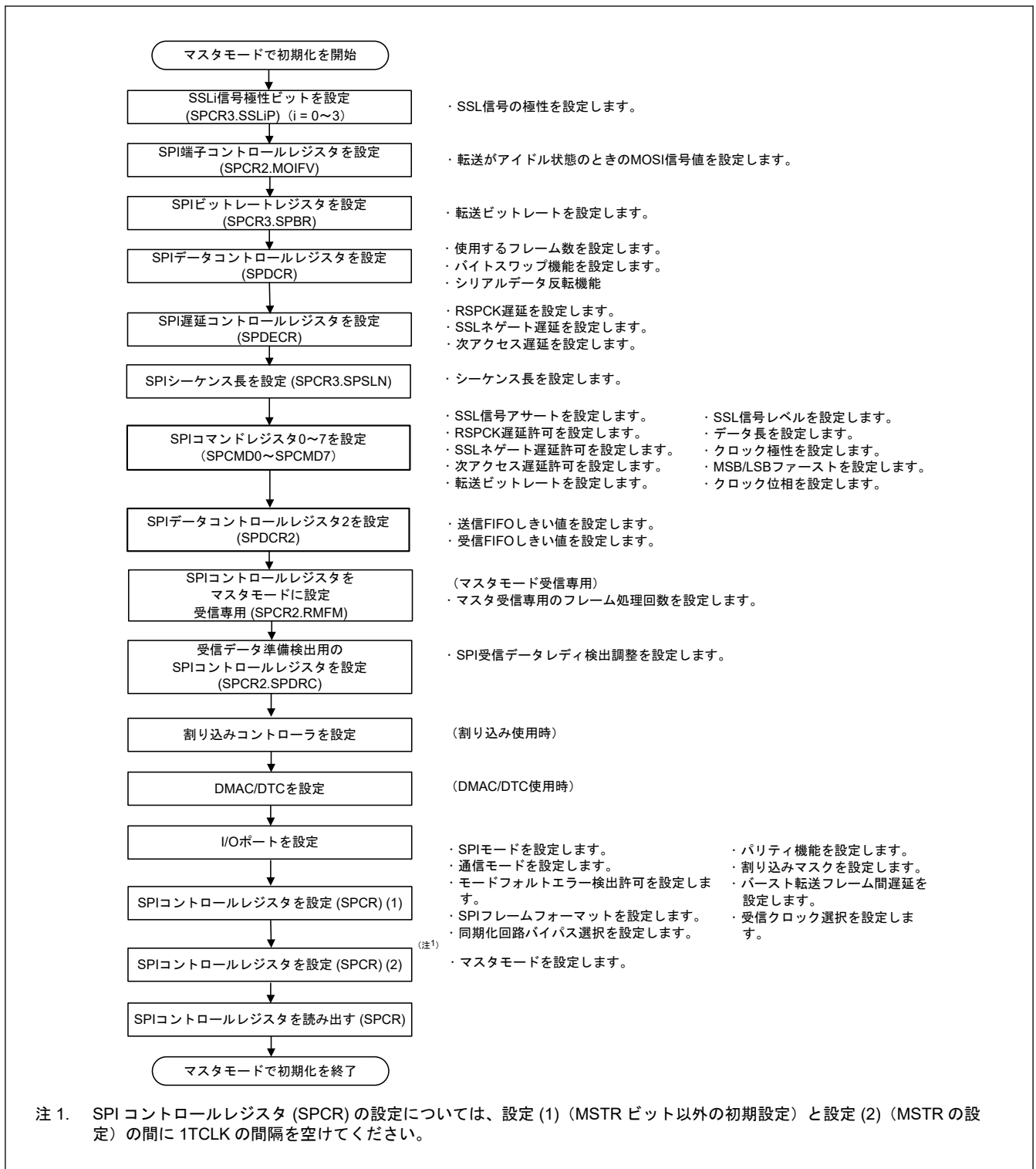
図 33.63 マスターモード時の SPI 動作の初期化フロー例
