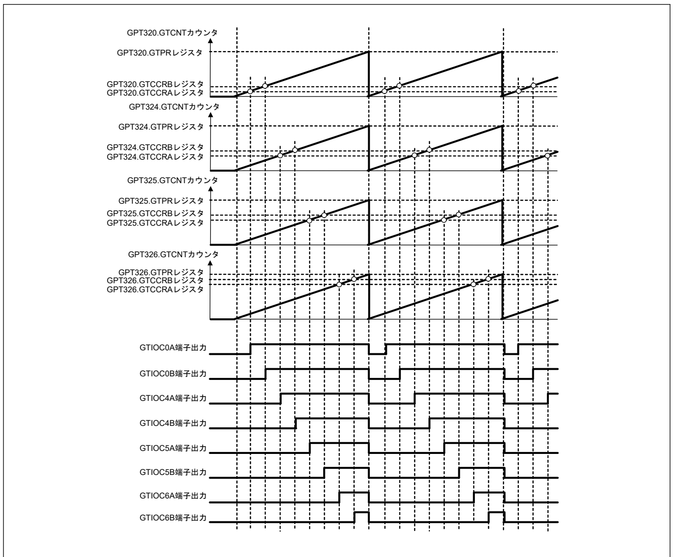
図 20.44 同期 PWM 出力例
