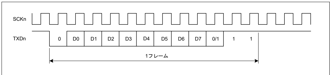
図 28.8 調歩同期式モードにおける出力クロックと送信データの位相関係 (CCR1.PE = 1、CCR3.CHR[1:0] = 10b、MP = 0、および STP = 1 の場合)
