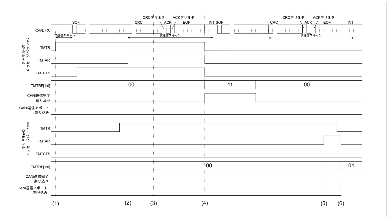
図 31.44 送信アボートの要求およびフラグビットのタイミング
