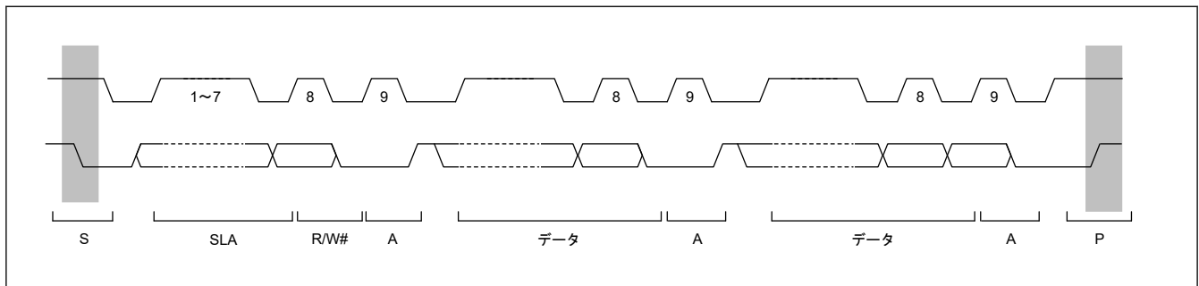
図 30.70 I 2 C バスタイミング (SLA = 7 ビットの場合)
