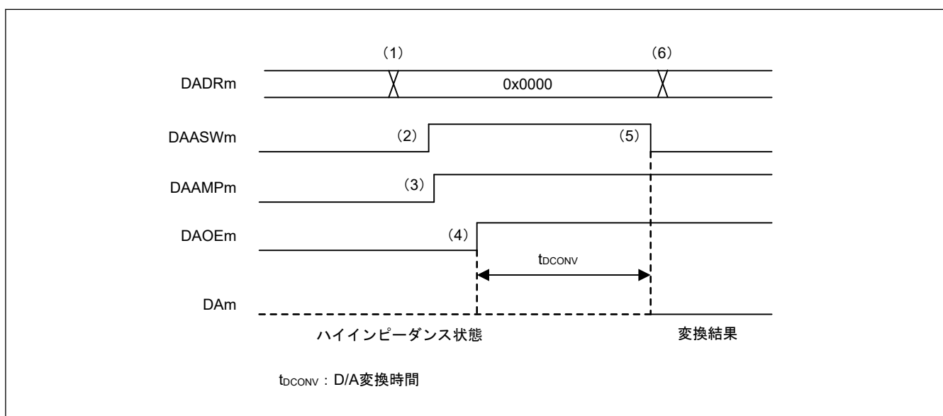
図 40.5 出力アンプを使用した DAC12 の初期化フロー例
