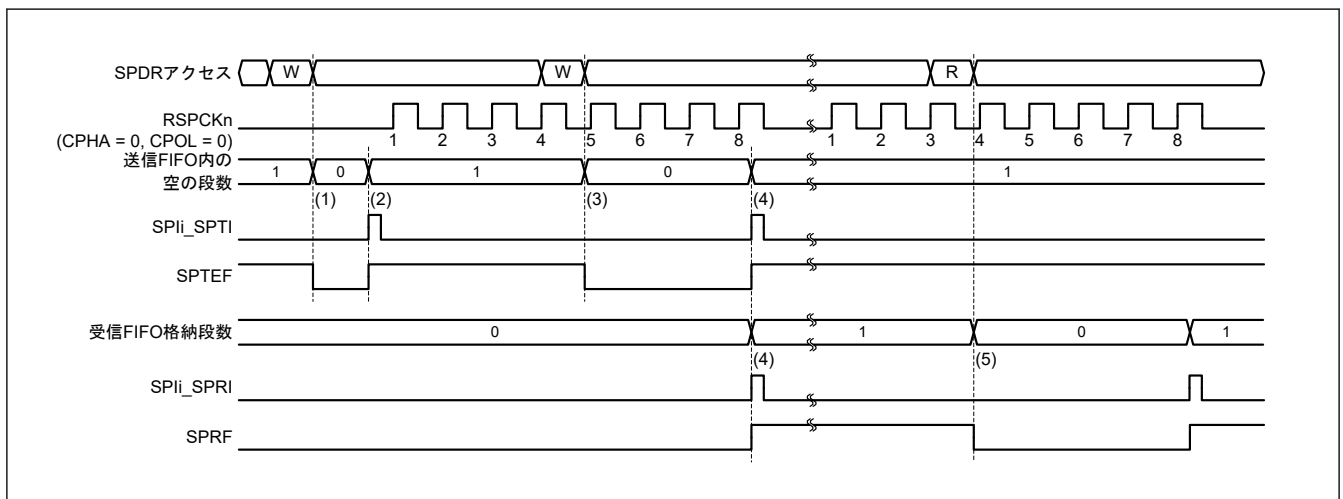
図 33.33 SPIi_SPTI、SPIi_SPRI 割り込みの動作例 (CPHA = 0、CPOL = 0)
