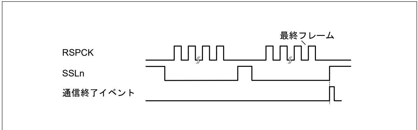
図 33.83 通信終了イベント出カタイミング (受信専用スレーブモード、Motorola SPI 動作)
