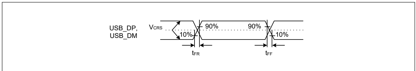
図 48.93 フルスピードモードにおける USB_DP、USB_DM の出力タイミング
