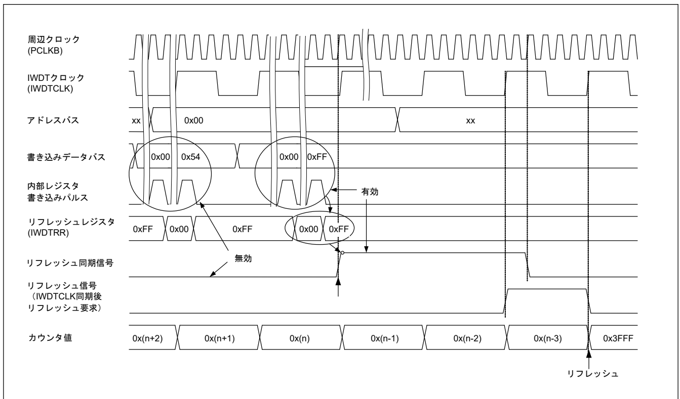
図 24.6 IWDT リフレッシュ動作波形 (IWDTCR.CKS[3:0] = 0000b, IWDTCR.TOPS[1:0] = 11b)
