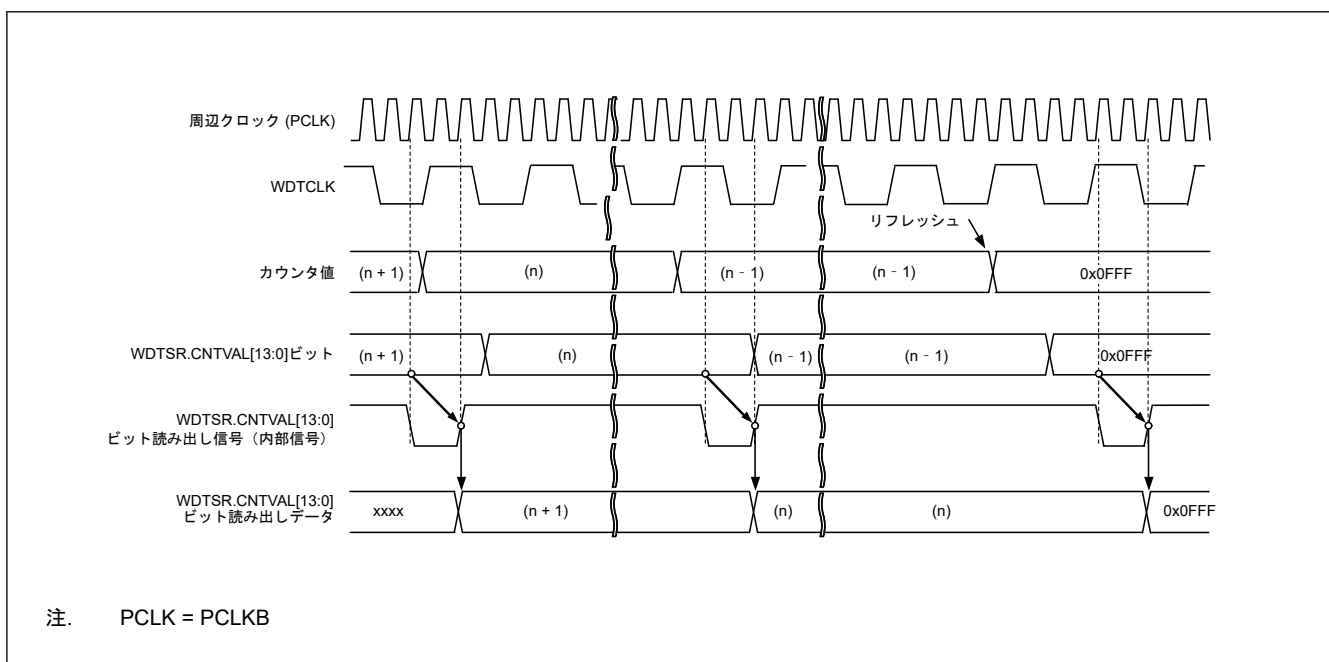
図 23.7 WDT ダウんカウンタ値の読み出し処理 (WDTCR.CKS[3:0] = 0x4、WDTCR.TOPS[1:0] = 01b の場合)
