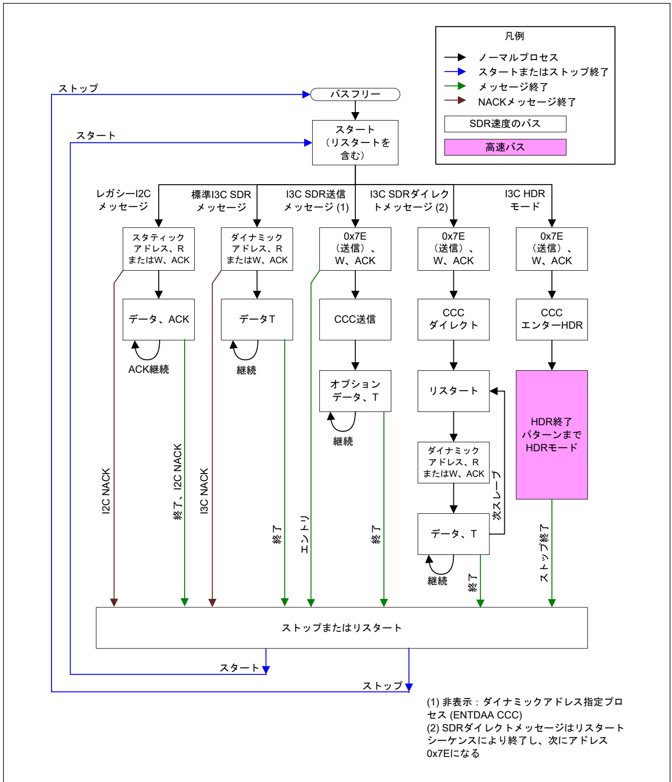
図 30.142 I3C 通信フロー
