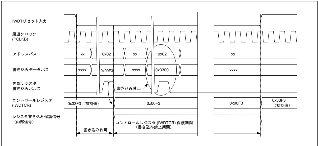
図 24.5 IWDTCR レジスタへの書き込みに対して生成される制御波形
