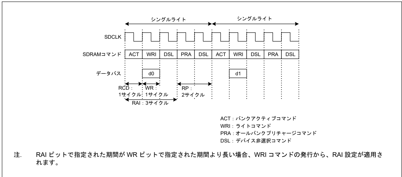
図 13.57 シングルライトタイミング例 (1)
