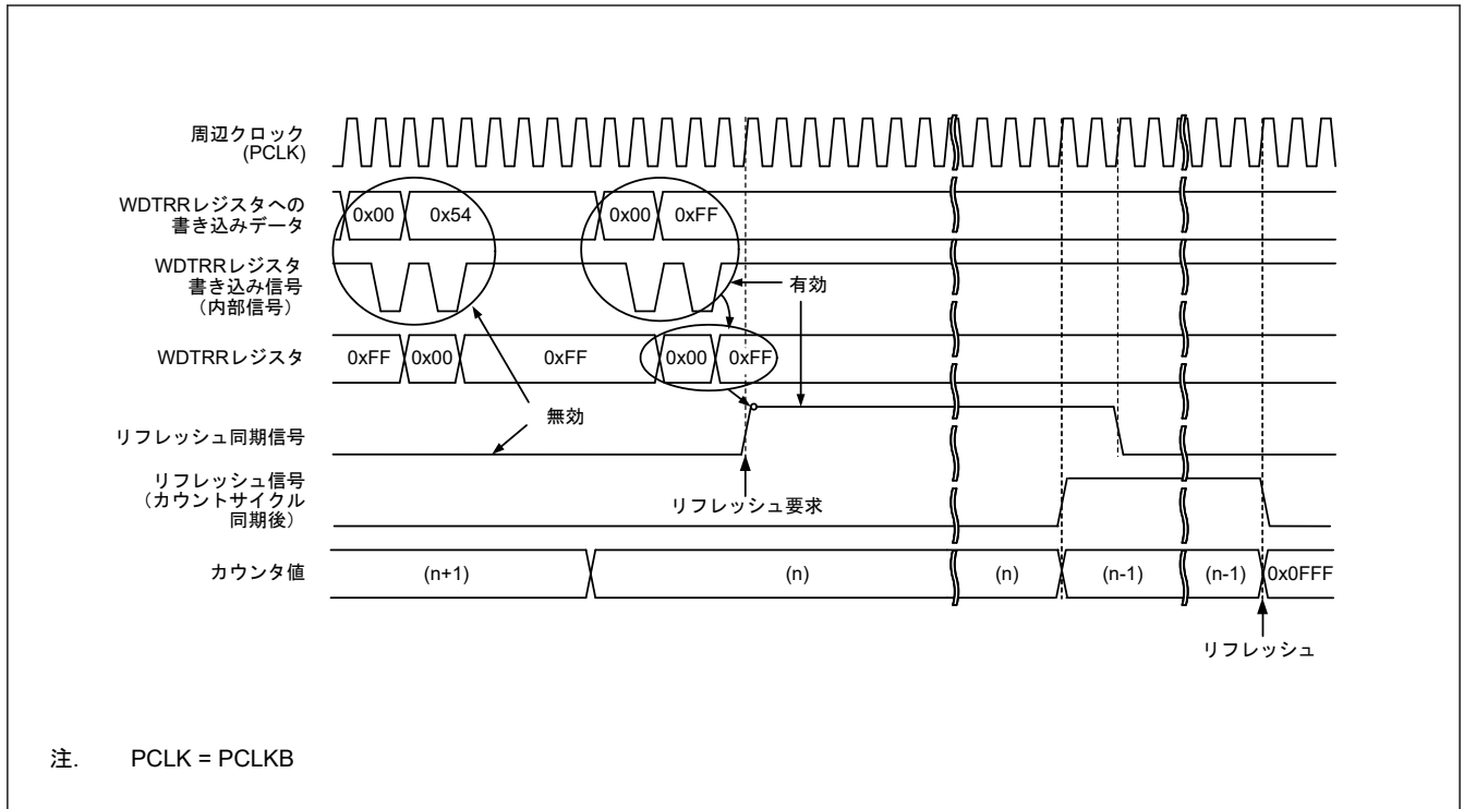
図 23.3 WDT リフレッシュ動作波形 (WDTCR.CKS[3:0] = 0x4、WDTCR.TOPS[1:0] = 01b の場合)
