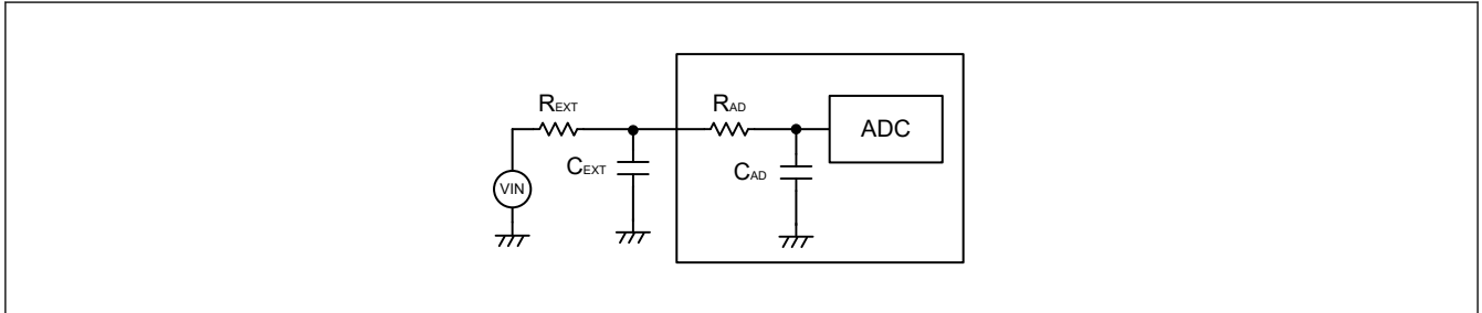
図 39.45 サンプル&ホールド回路の簡略図
