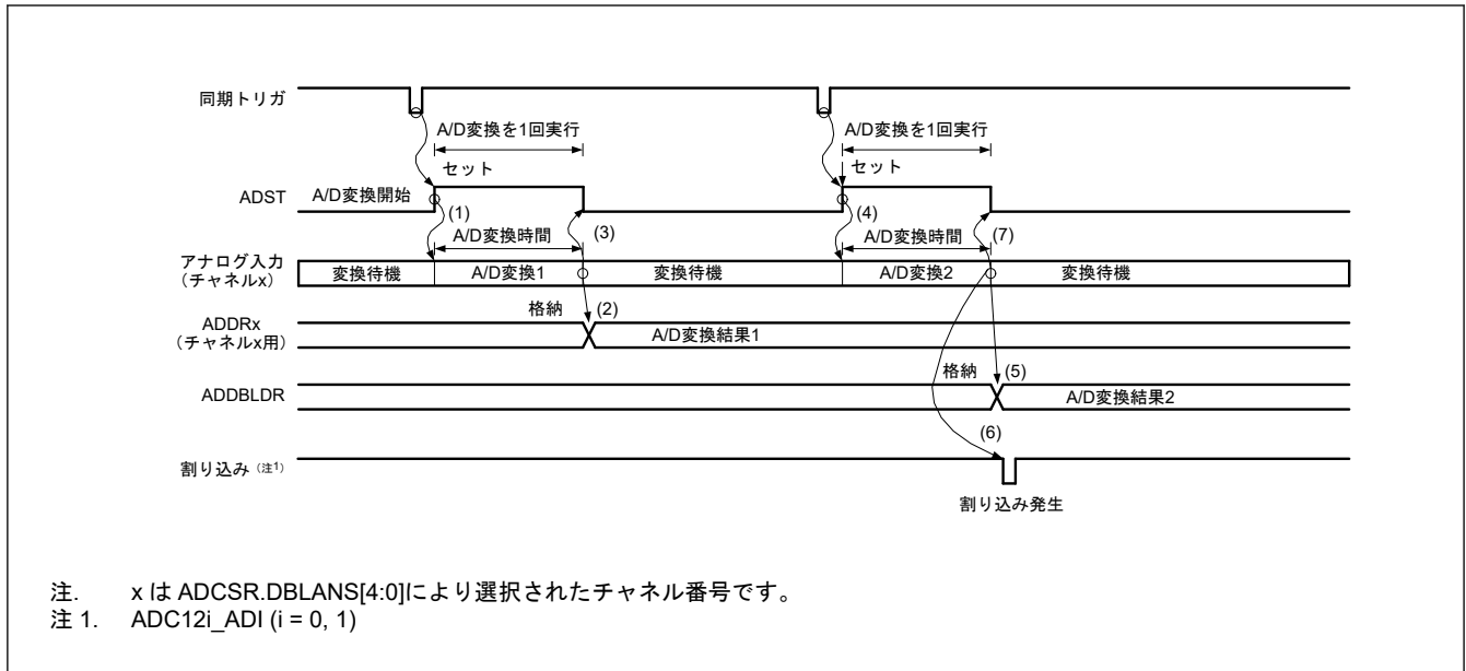
図 39.15 シングルスキャンモードの動作例 (ダブルトリガモード選択、アナログ入力 (チャンネル x) を 2 重化)
