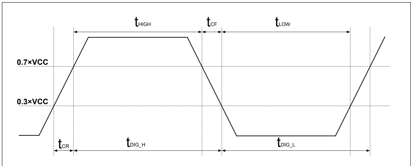
図 48.68 t_{DIG\_H} 、 t_{DIG\_L}
