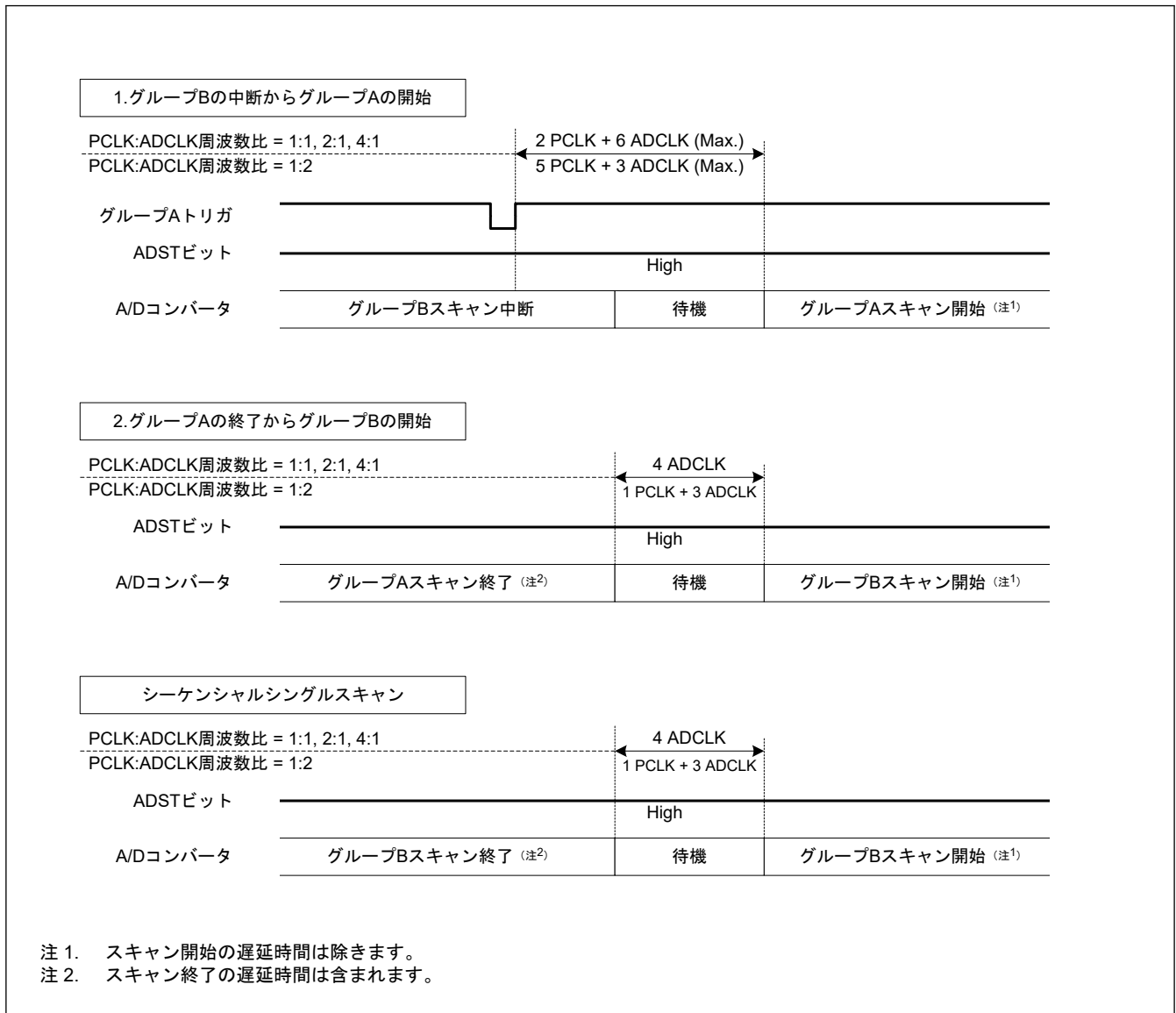
図 39.37 グループ優先制御における動作でのスキャンの中断/開始タイミング図
