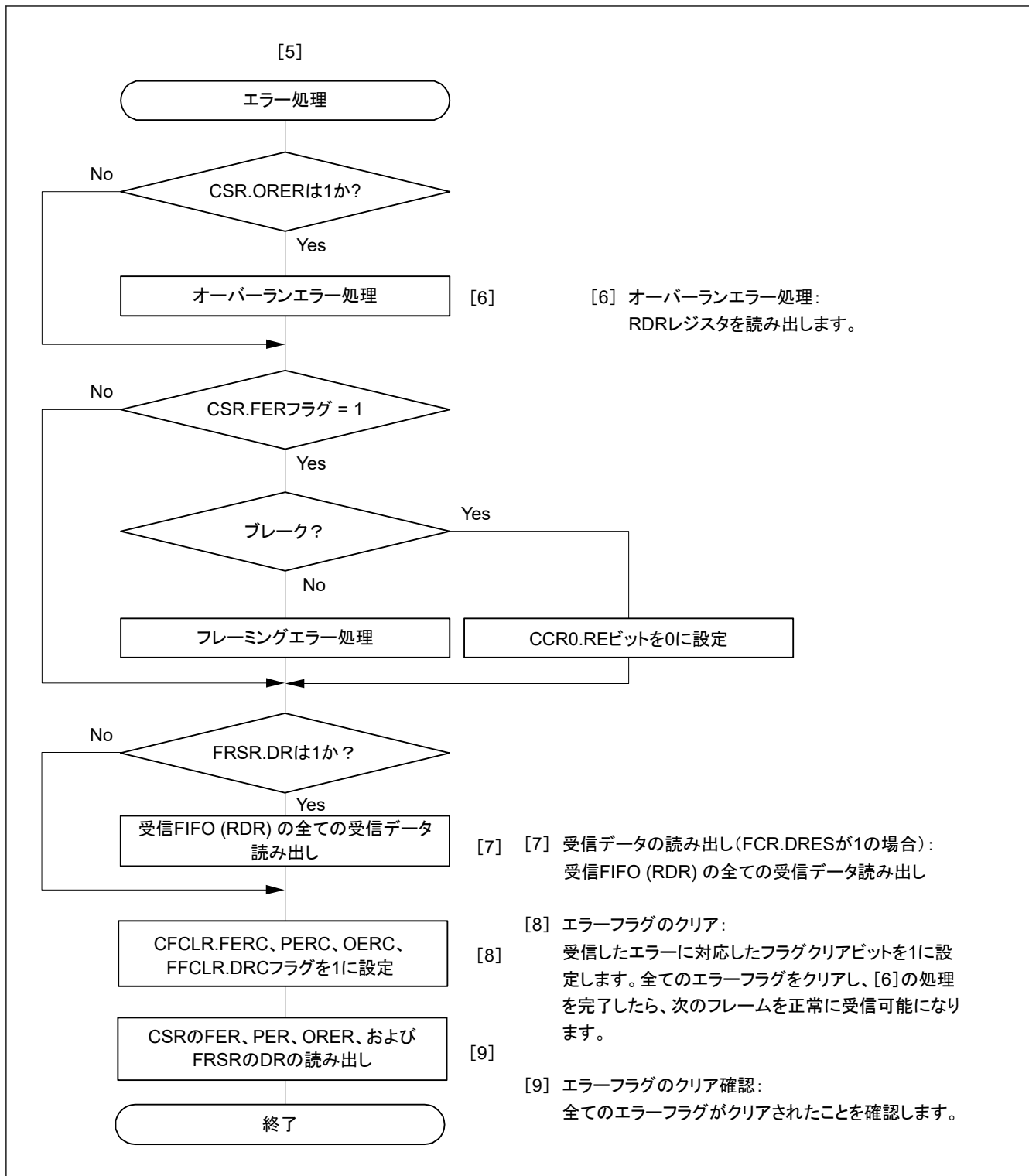
図 28.44 マルチプロセッサモードにおけるシリアル受信のフローチャート例 (2) (FIFO 選択時)
