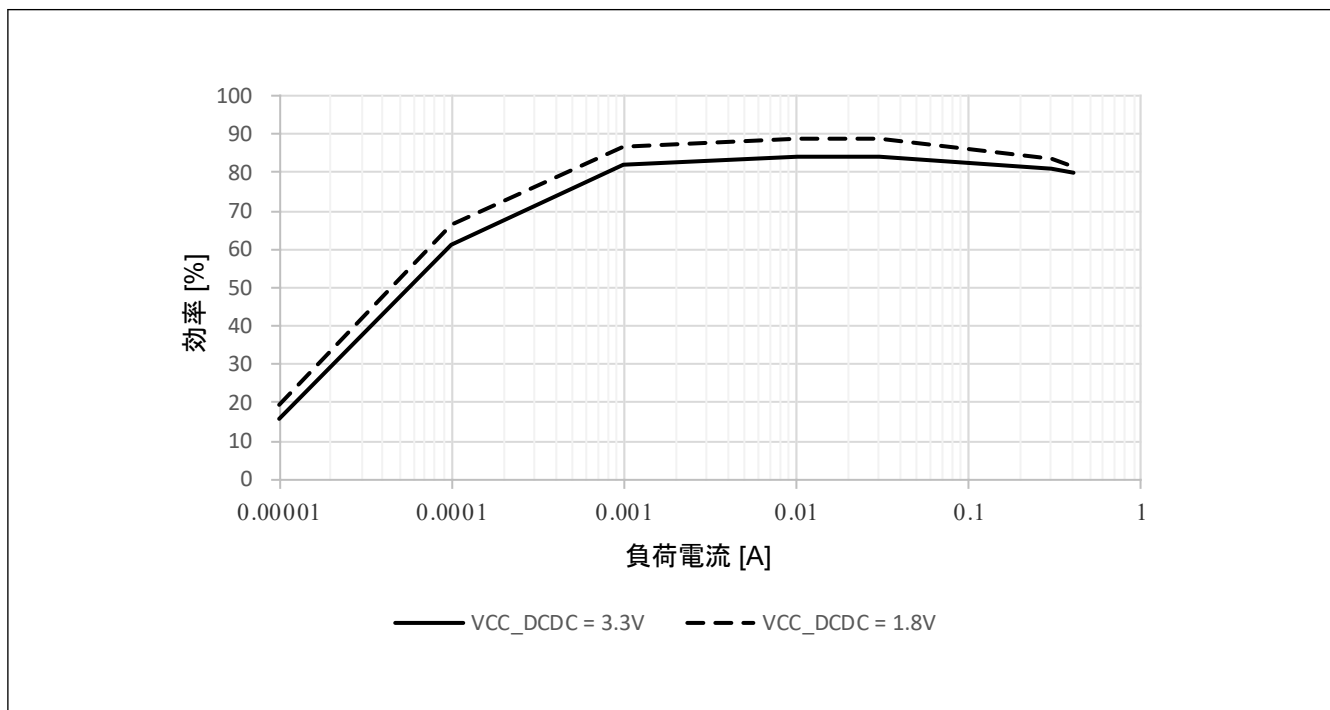
図 48.11 Low-speed モードおよびソフトウェアスタンバイモード、Tj = 25°Cにおける標準 DCDC 効率 (%) と負荷電流 (A)
