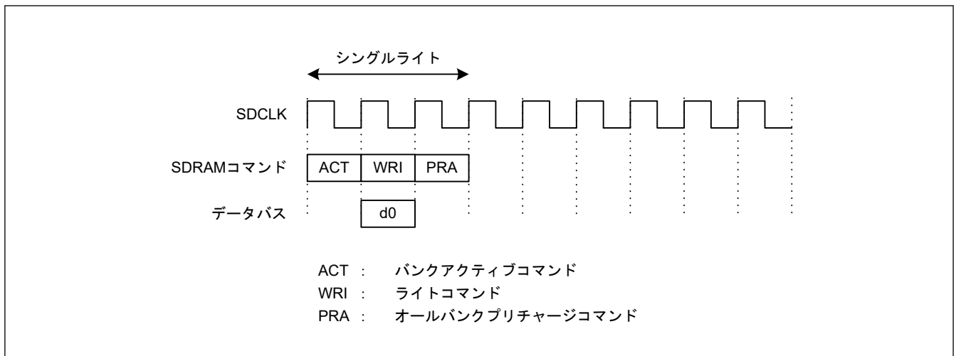
図 13.45 シングルライトのタイミング例 (最短のタイミングを設定したとき)
