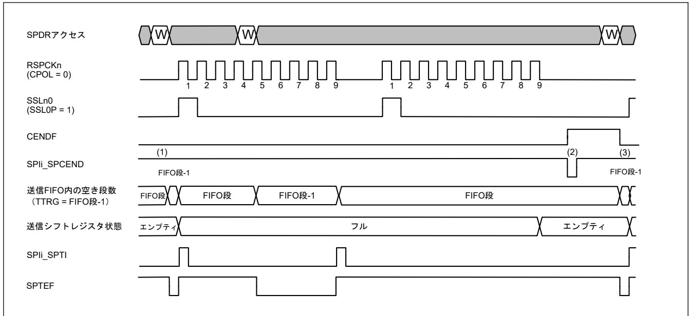
図 33.41 通信終了割り込み動作例 (SPI 動作/TI-SSP 時の送受信/送信専用スレーブモード)
