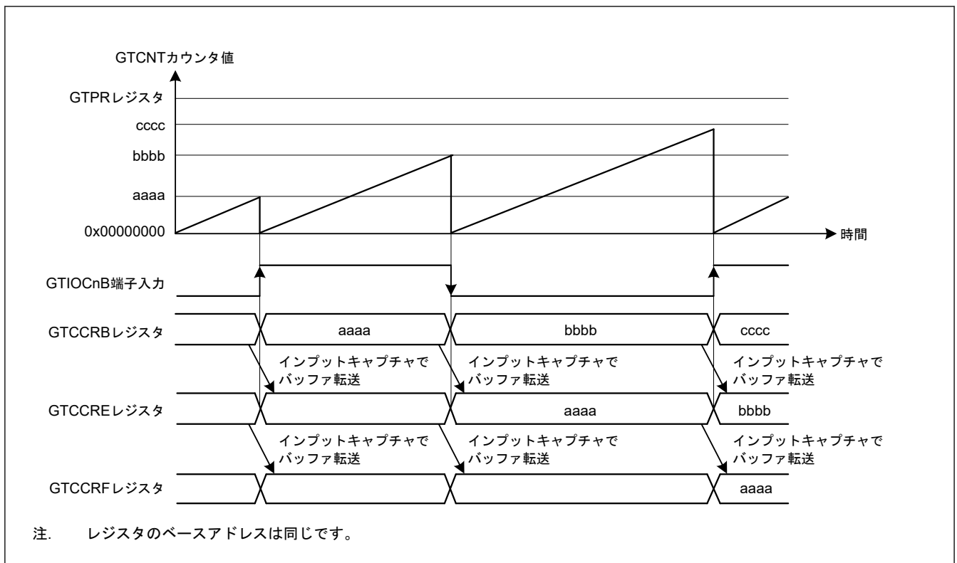
図 20.17 GTCCRA および GTCCRB レジスタのダブルバッファ動作例 (GTIOcNB 端子入力の両エッジでインプットキャプチャ、のこぎり波でアップカウント、GTIOcNB 端子入力の両エッジで GTCNT カウンタクリアの場合)
