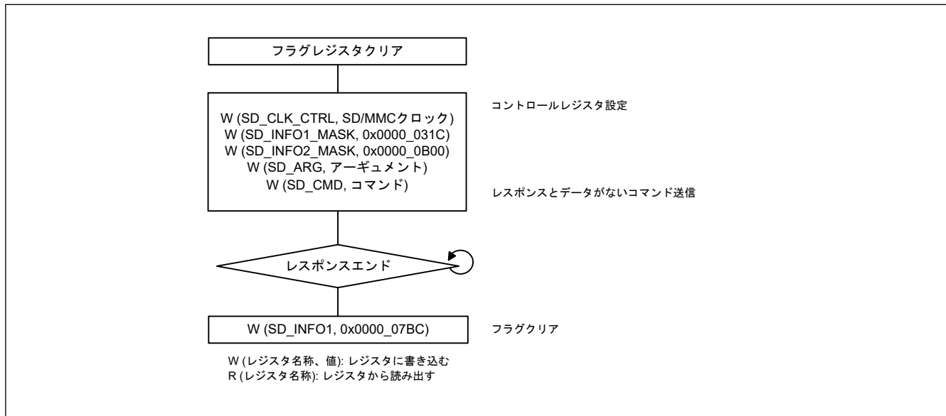
図 34.9 レスポンスまたはデータがないコマンドのフロー例
