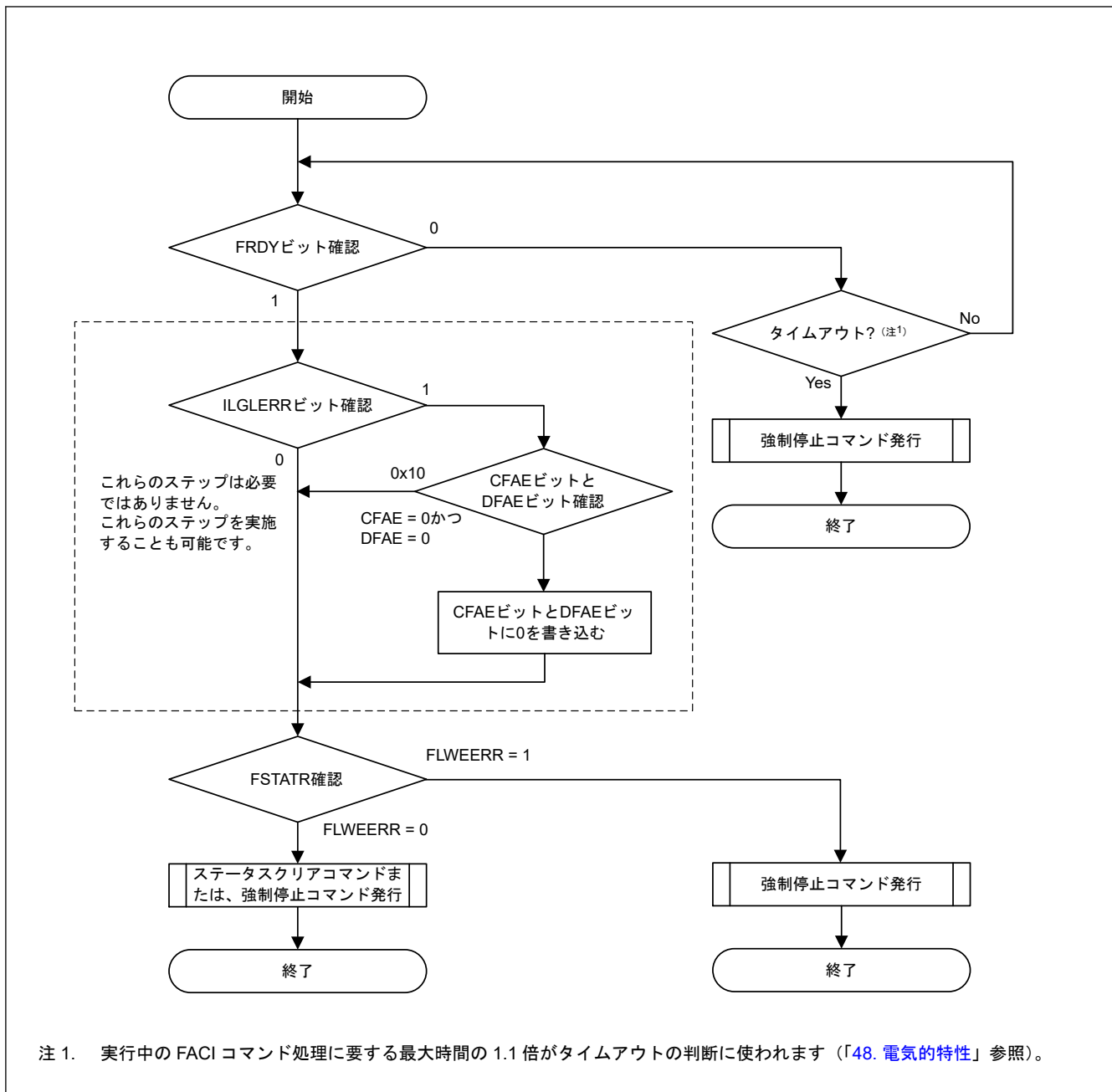
図 46.13 コマンドロック状態からの復帰フロー
