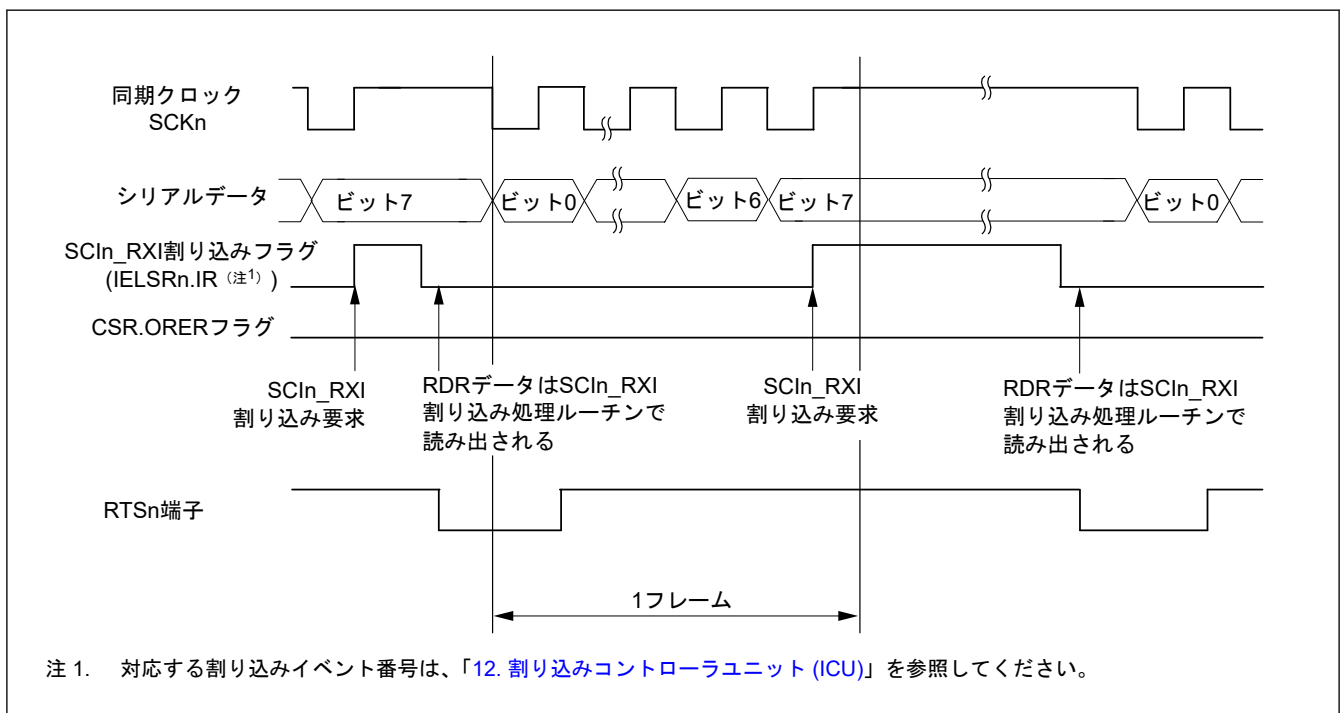
図 28.68 クロック同期式モードにおけるシリアル受信の動作例 (2) (RTS 機能を使用する場合)
