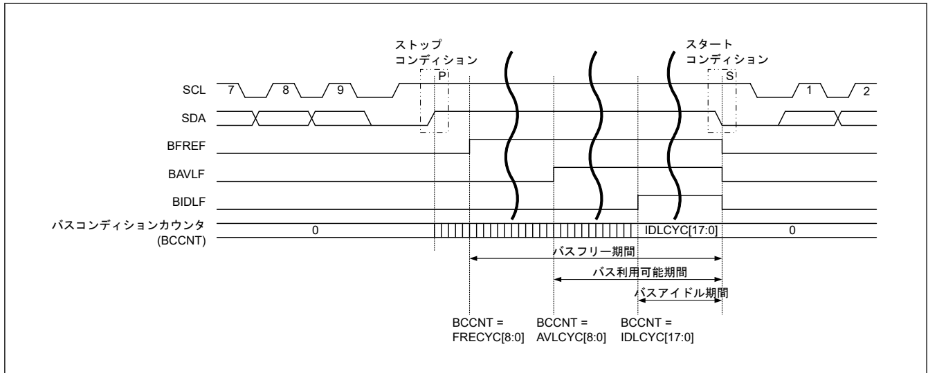
図 30.78 バス状態
