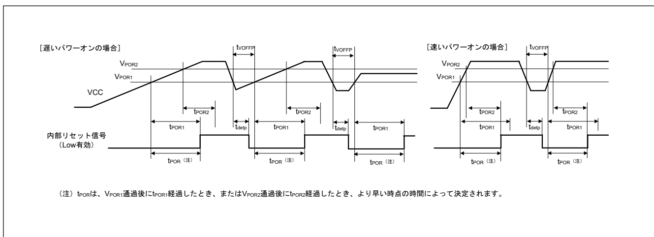
図 48.97 パワーオンリセットタイミング
