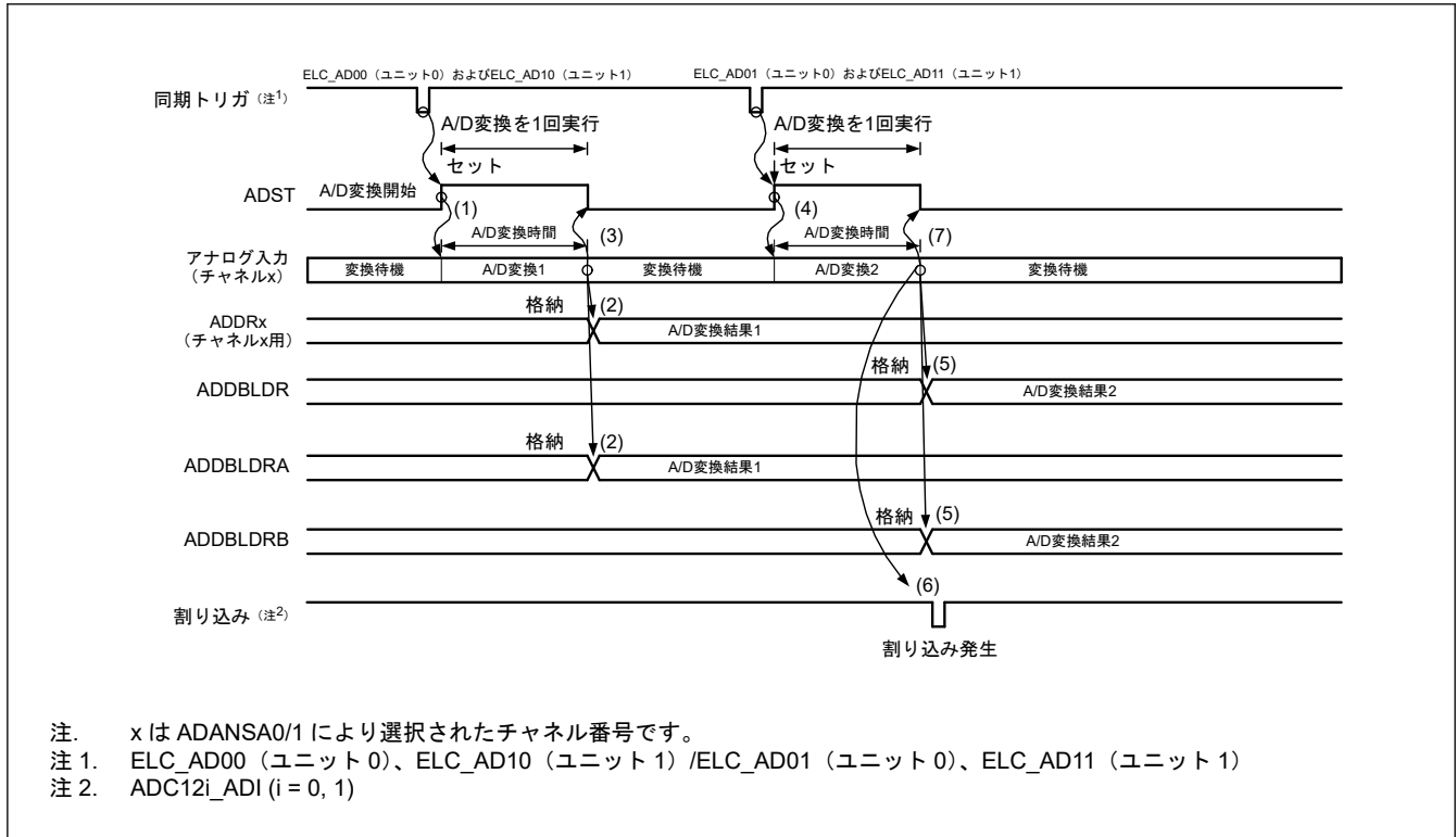
図 39.16 アナログ入力 (チャンネル x) と ELC_AD00 (ユニット 0)、ELC_AD10 (ユニット 1) /ELC_AD01 (ユニット 0)、ELC_AD11 (ユニット 1) の重複選択時のダブルトリガモード拡張動作例
