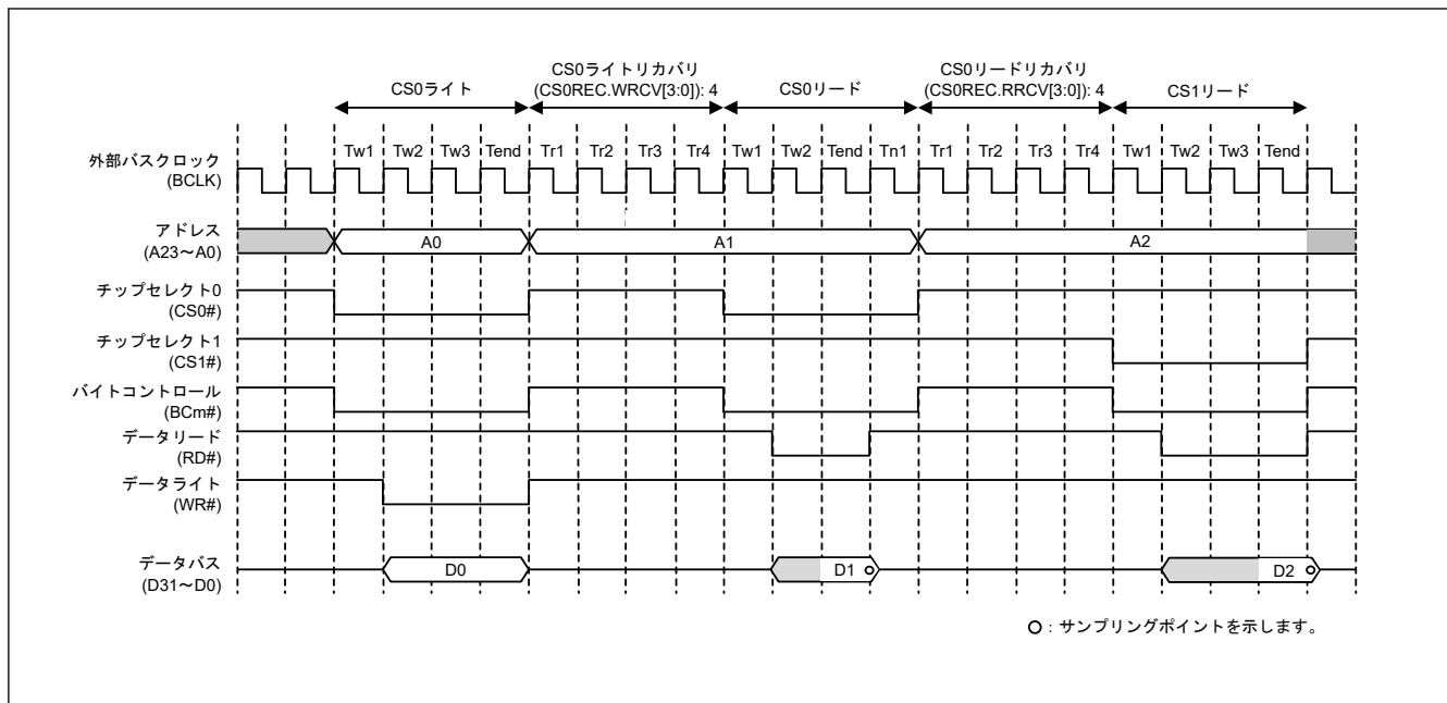
図 13.29 セパレートバスインタフェース時のリカバリサイクルの挿入例 (m = 0~3)
