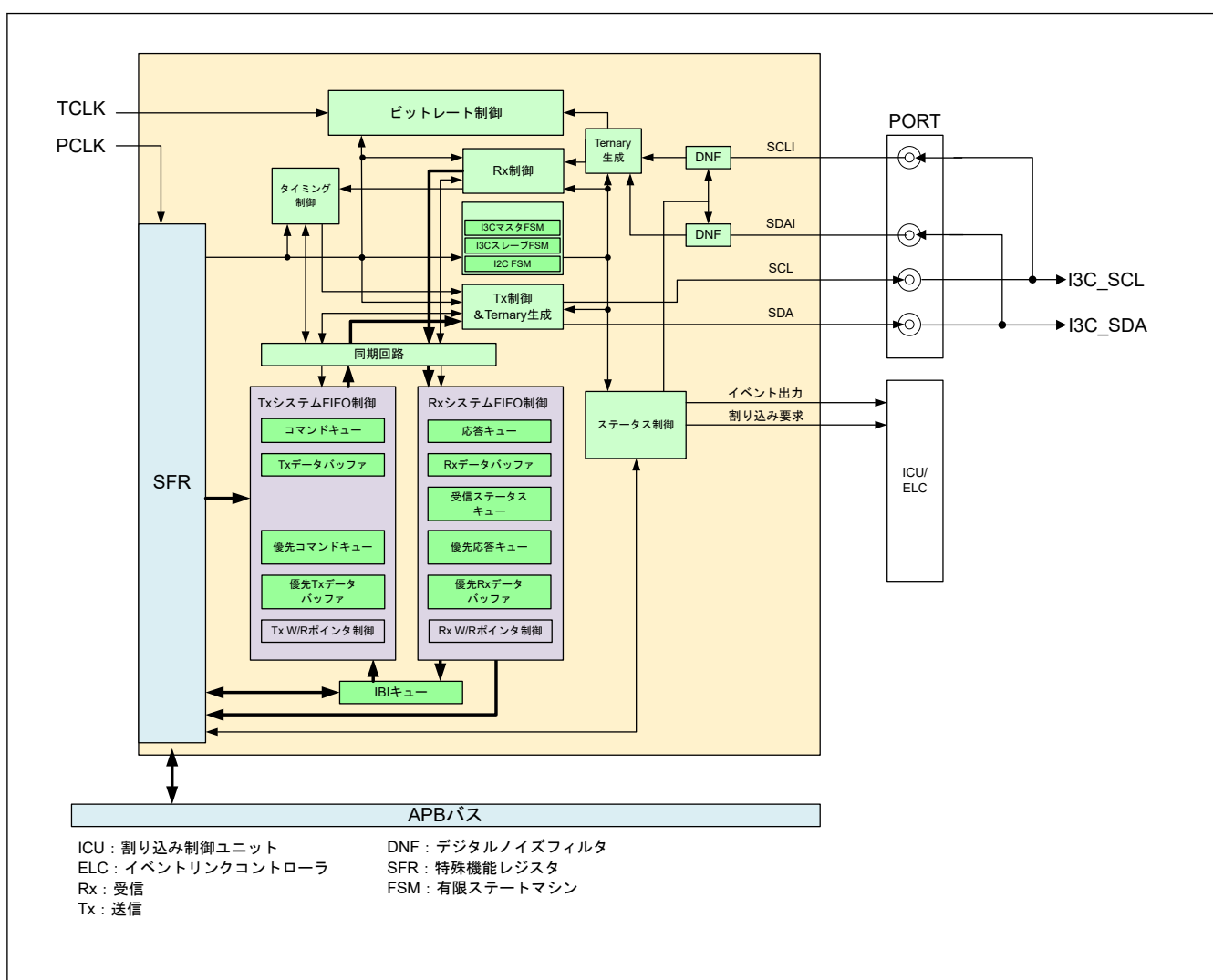
図 30.1 I3C ブロック図
