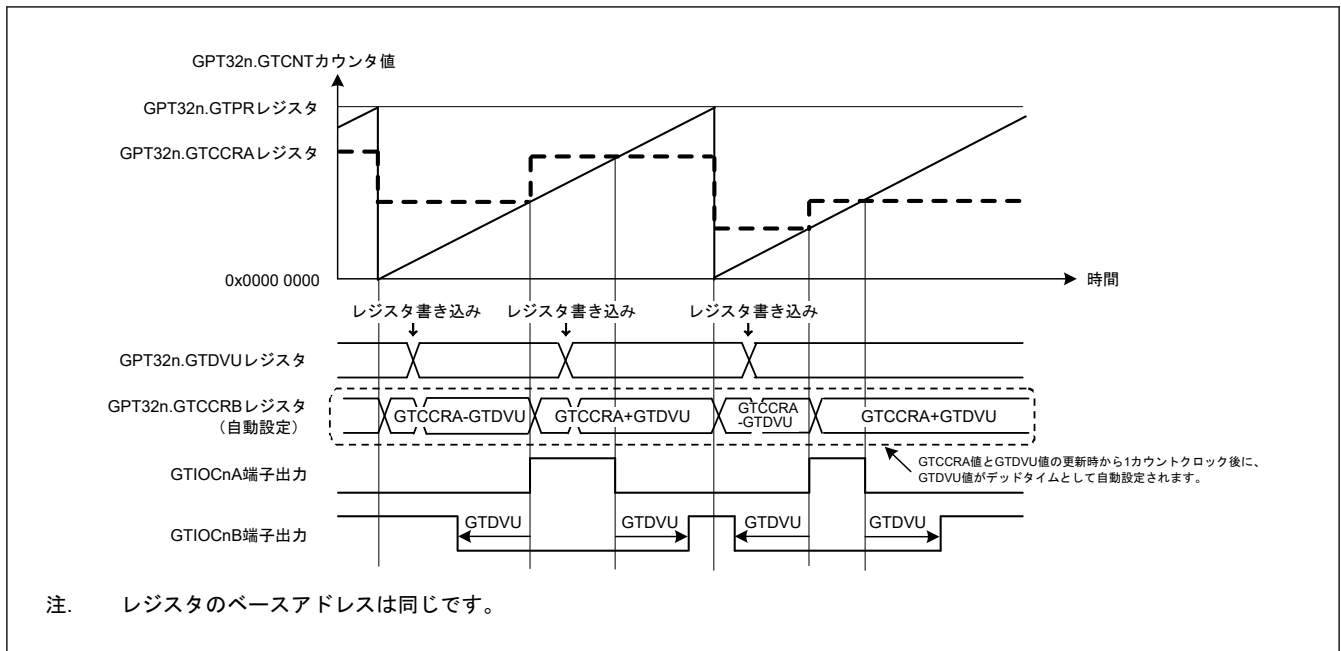
図 20.26 デッドタイム自動設定機能の動作例（のこぎり波ワンショットパルスモード、アップカウント、アクティブ High の場合）
