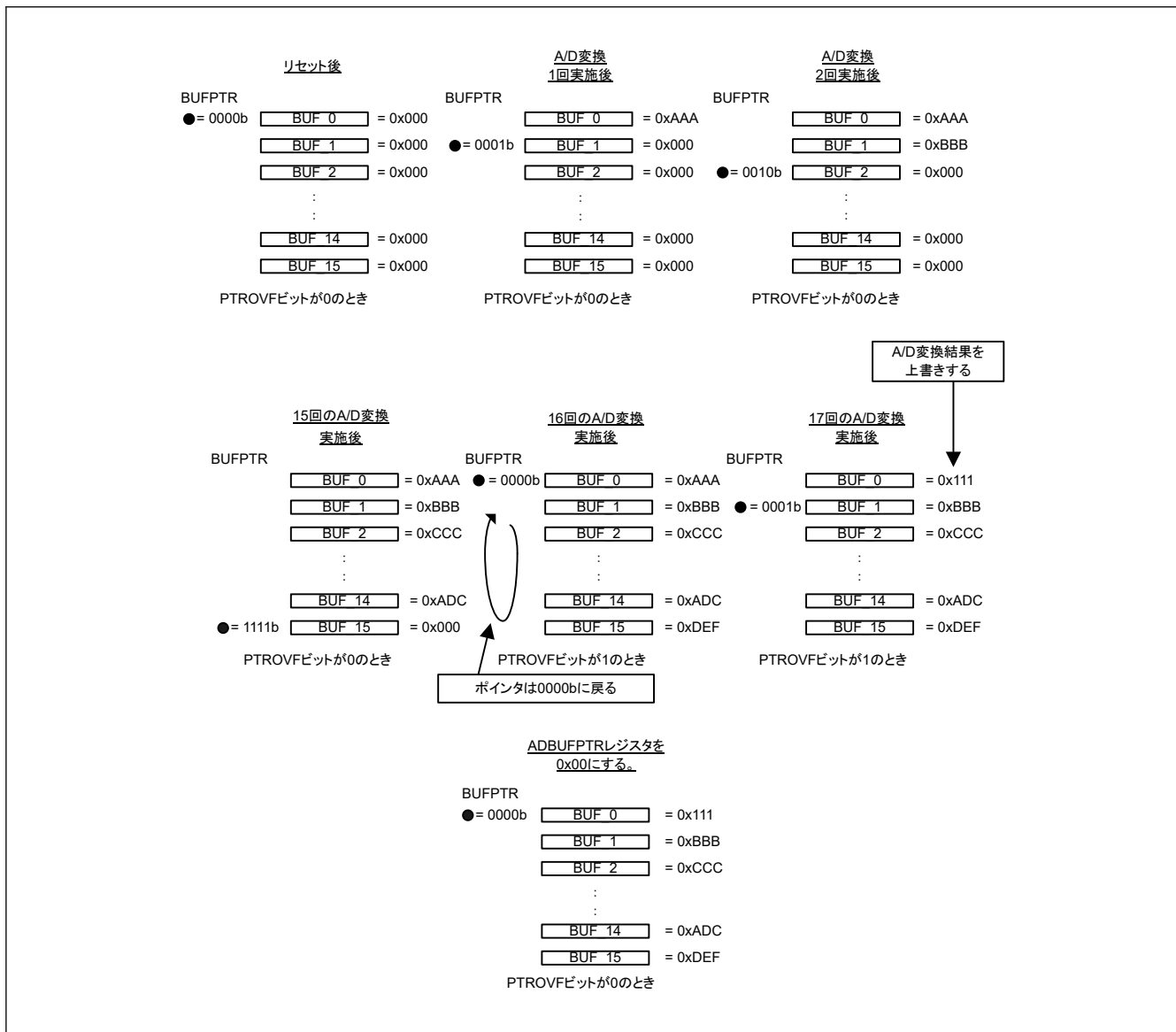
図 39.42 データバッファ、ポインタ、およびオーバーフローフラグの動作概略図
