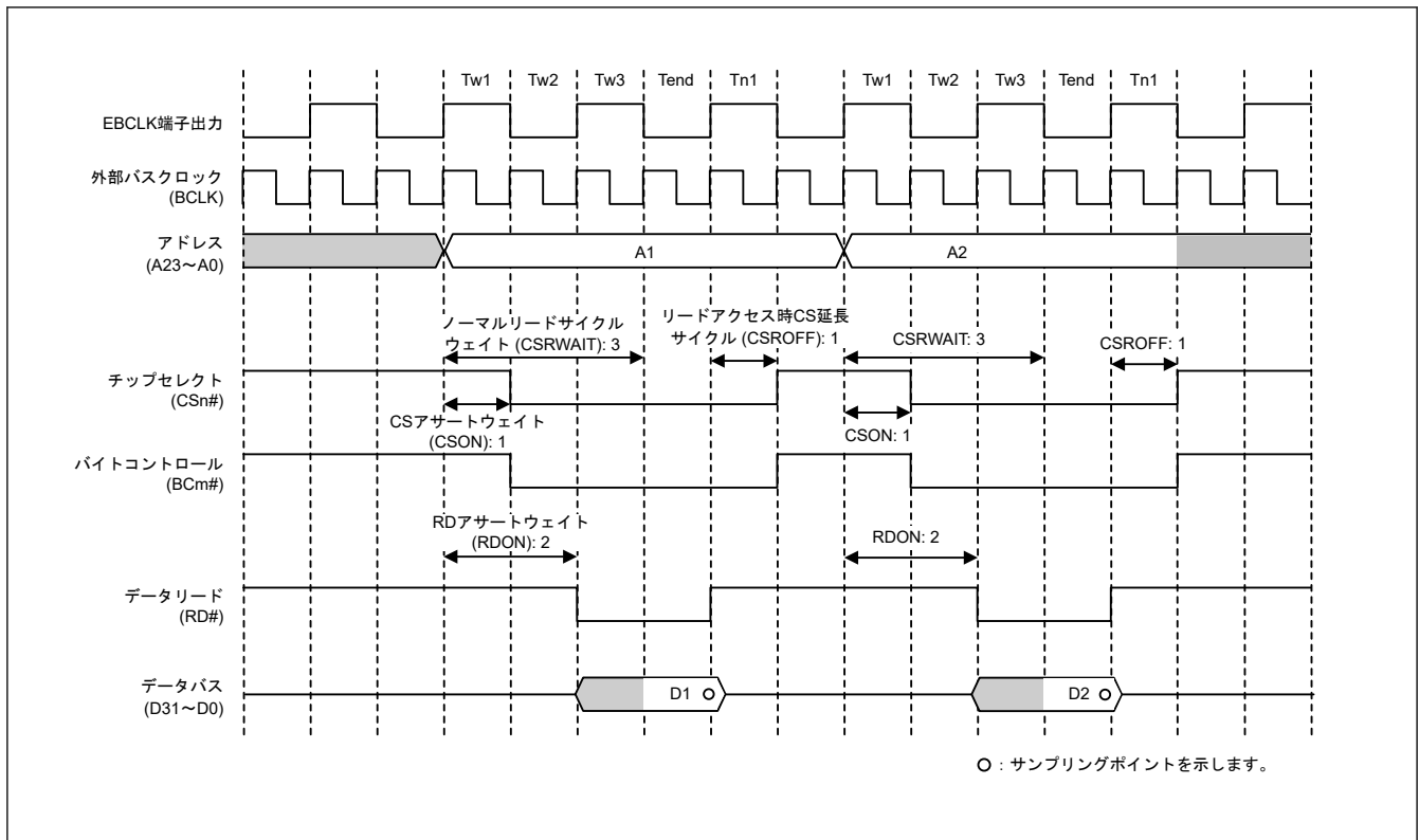
図 13.11 ノーマルリードアクセスの動作例 (EBCLK 端子出力選択ビットで BCLK の 2 分周を設定した場合) (n = 0~7, m = 0~3)
