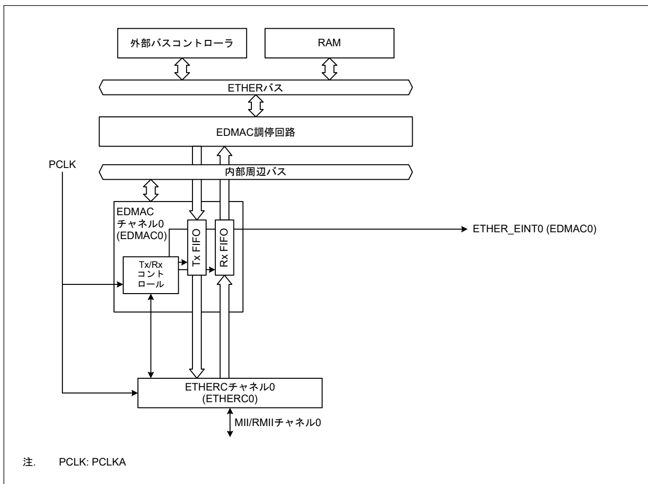
図 26.1 EDMAC の構成
