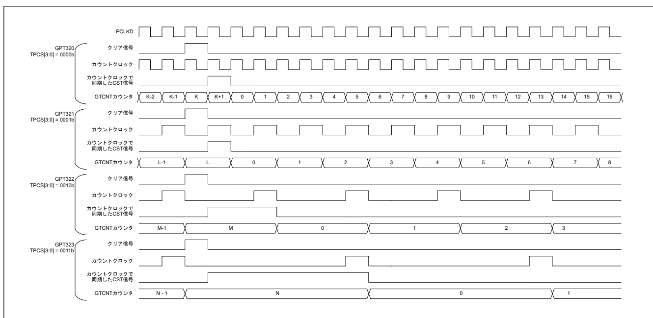
図 20.42 ソフトウェアによる同時クリアの動作例 (異なるカウント周期)
