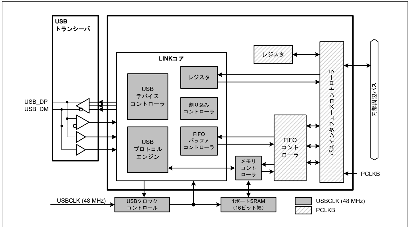
図 27.1 USBFS のブロック図
