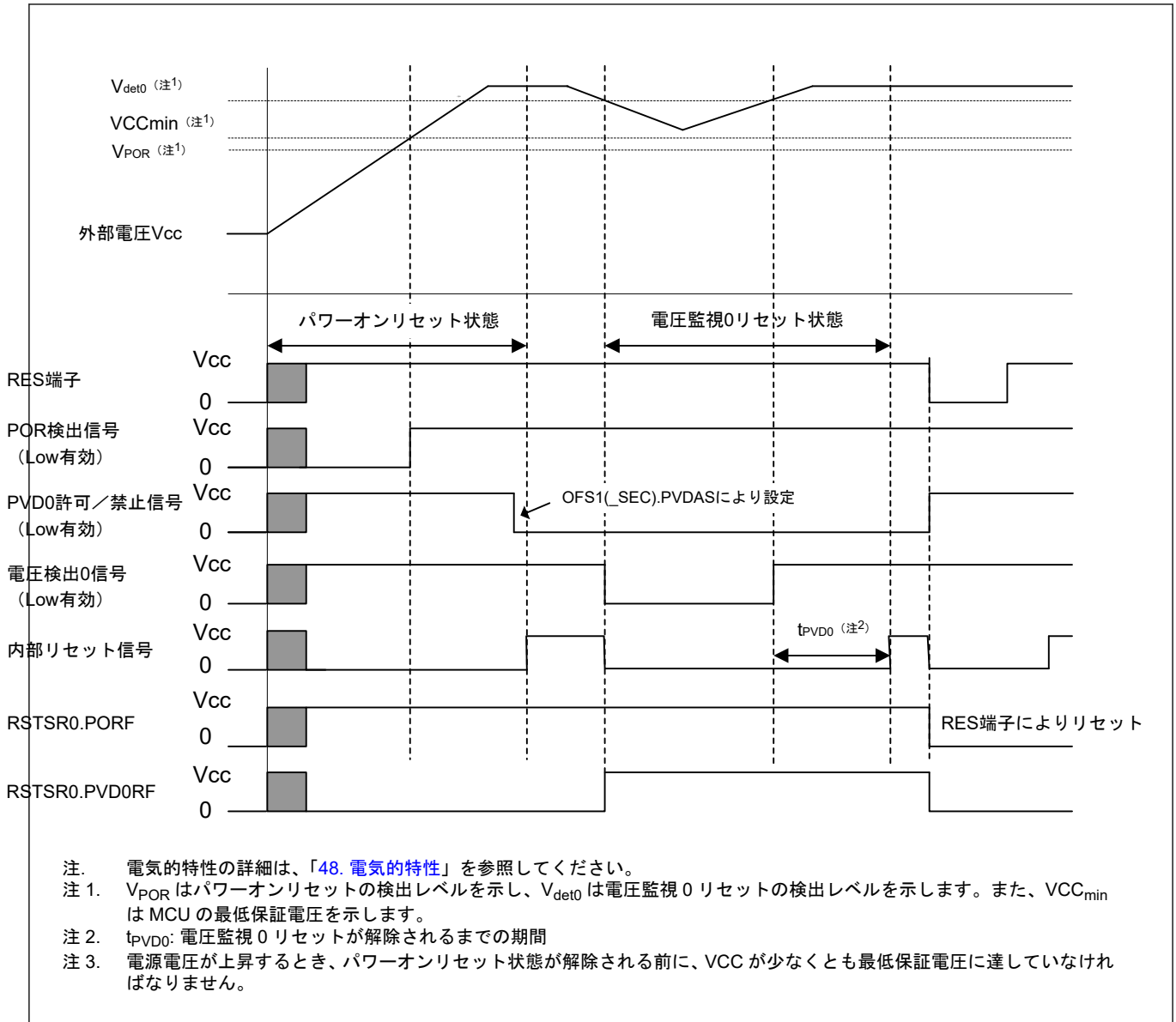
図 7.3 電圧監視 0 リセットの動作例
