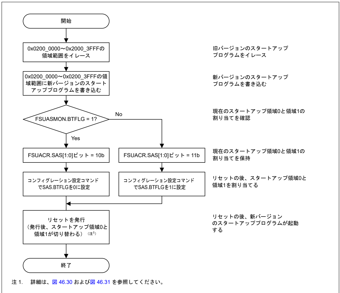
図 46.32 スタートアッププログラムプロテクションの概念 (セキュアエアリアスの場合)
