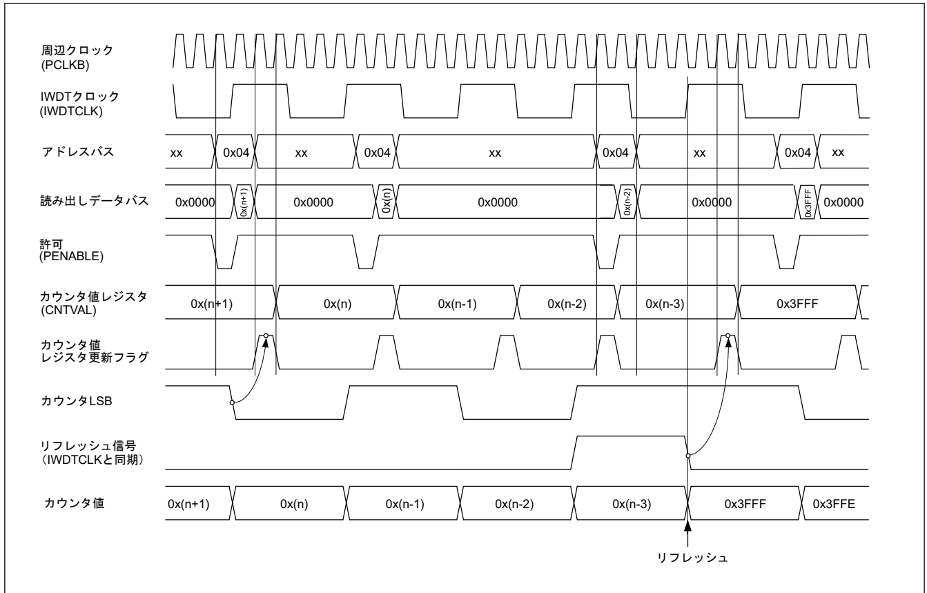
図 24.8 IWDT カウンタ値の読み出し処理 (IWDTCR.CKS[3:0] = 0000b、IWDTCR.TOPS[1:0] = 11b の場合)
