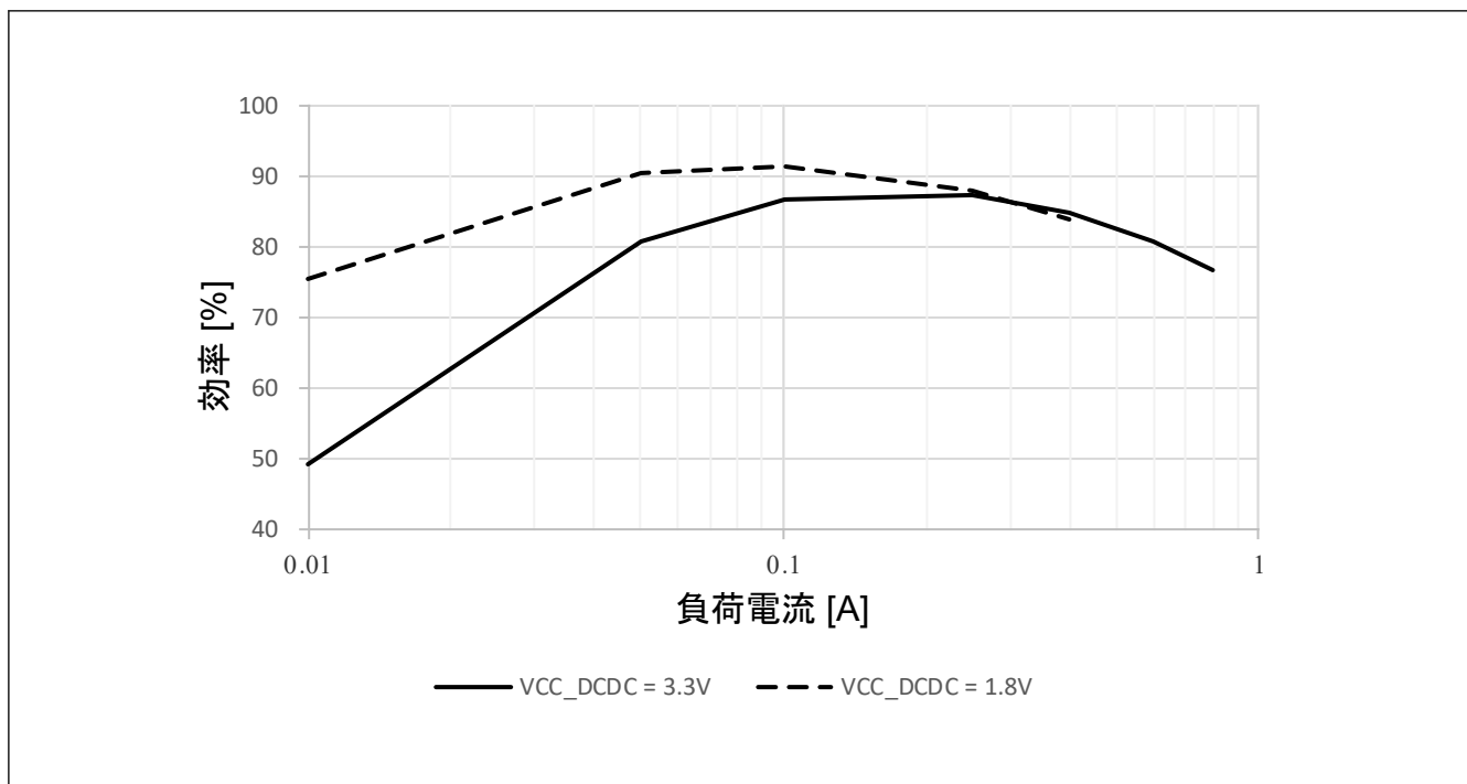
図 48.9 High-speed モード、T j = 25°Cにおける標準 DCDC 効率 (%) と負荷電流 (A)
