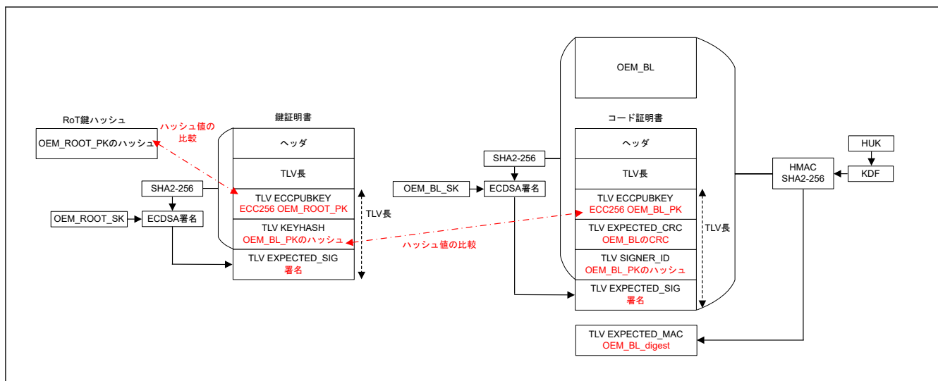
図 37.13 検証構成と証明書の形式
