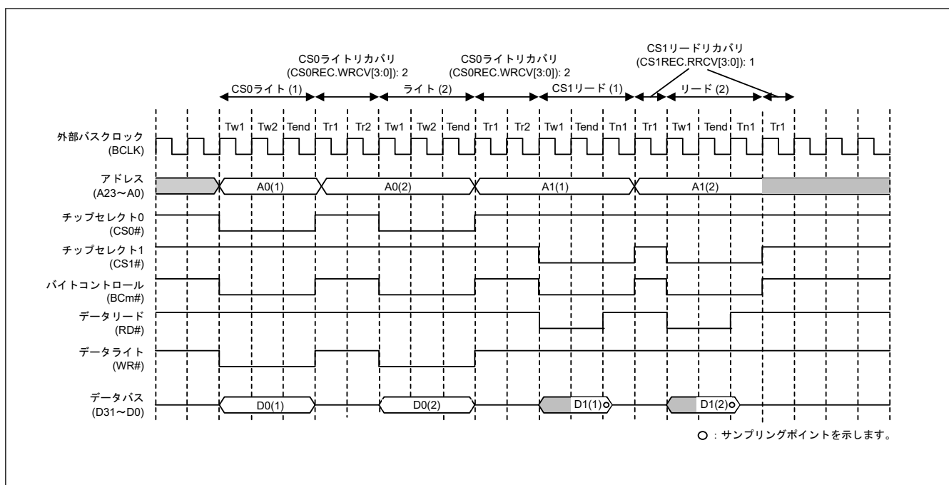
図 13.30 バスアクセスが分割された場合のリカバリサイクルの挿入例 (セパレートバスインタフェースによるノーマルアクセスの場合) (m = 0~3)
