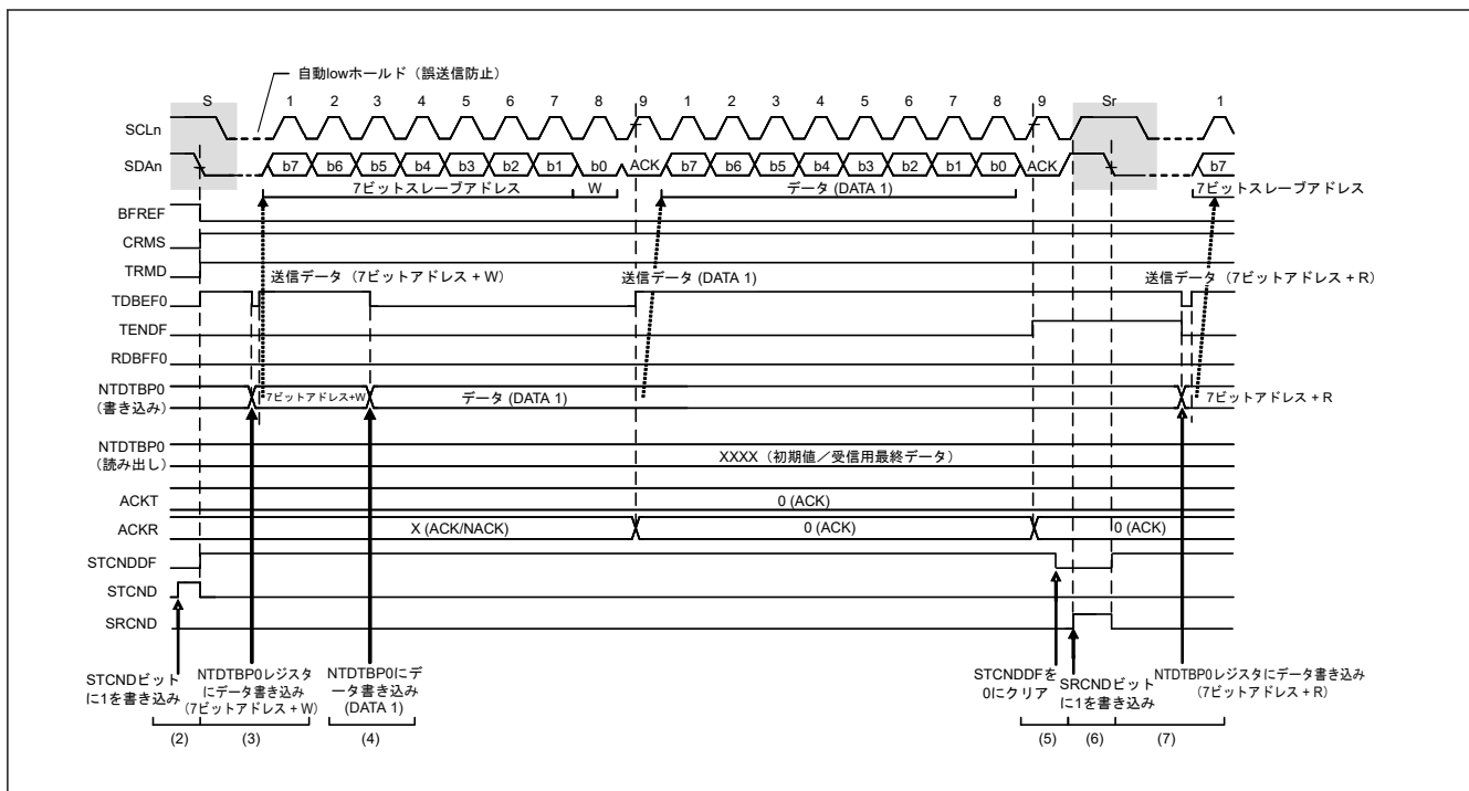
図 30.80 マスタ送信後の繰り返しのスタートコンディション発行タイミング
