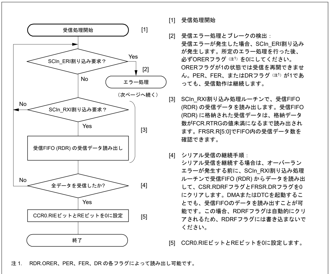
図 28.24 調歩同期式モードにおけるシリアル受信のフローチャート例 (FIFO 選択、アドレス一致検出有効時) (1)
