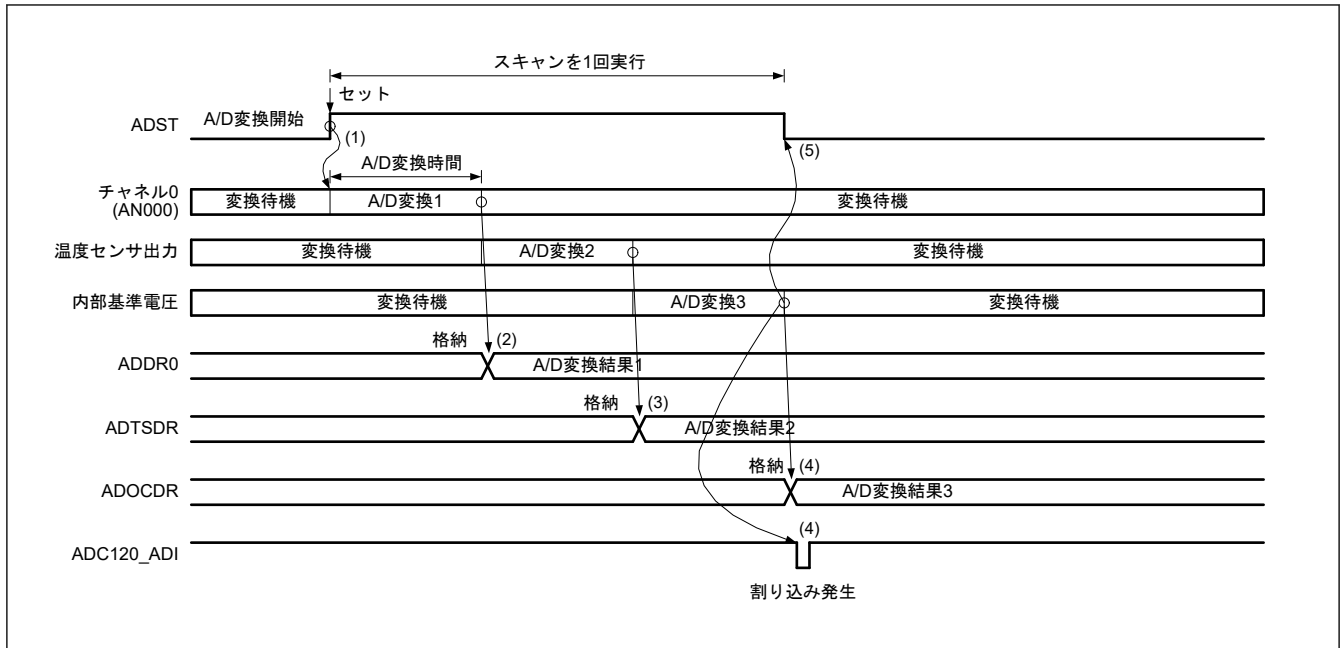
図 39.14 シングルスキャンモードの基本動作例 (AN000、温度センサ出力または内部基準電圧選択時)
