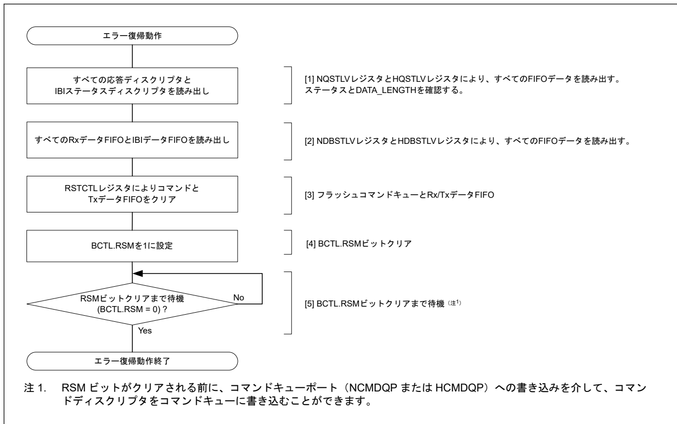
図 30.122 I3C マスタのエラー復帰動作フローの例
