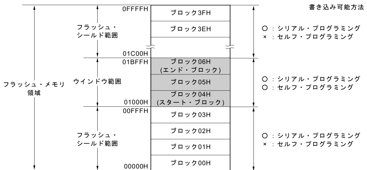
図30-11 フラッシュ・シールド・ウインドウの設定例 (対象デバイス：R5F104LE, スタート・ブロック：04H, エンド・ブロック：06Hの場合)
