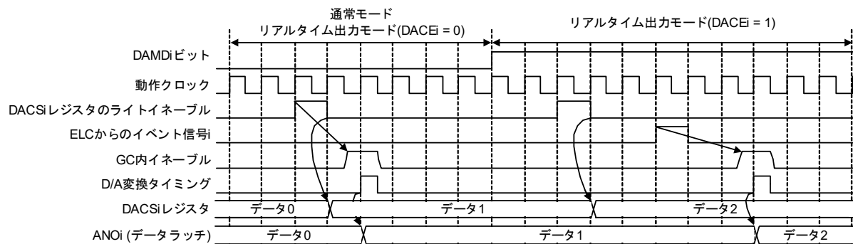
図15-5 D/A変換値の出カタイミング
