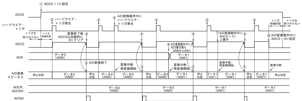
図14 - 28 ハードウェア・トリガ・ウエイト・モード(セレクト・モード, ワンショット変換モード)動作タイミング例
