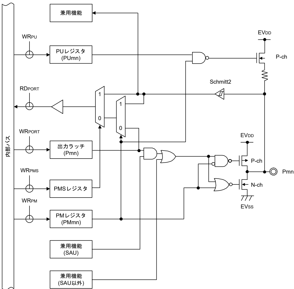
図2-7 端子タイプ7-1-3の端子ブロック図
