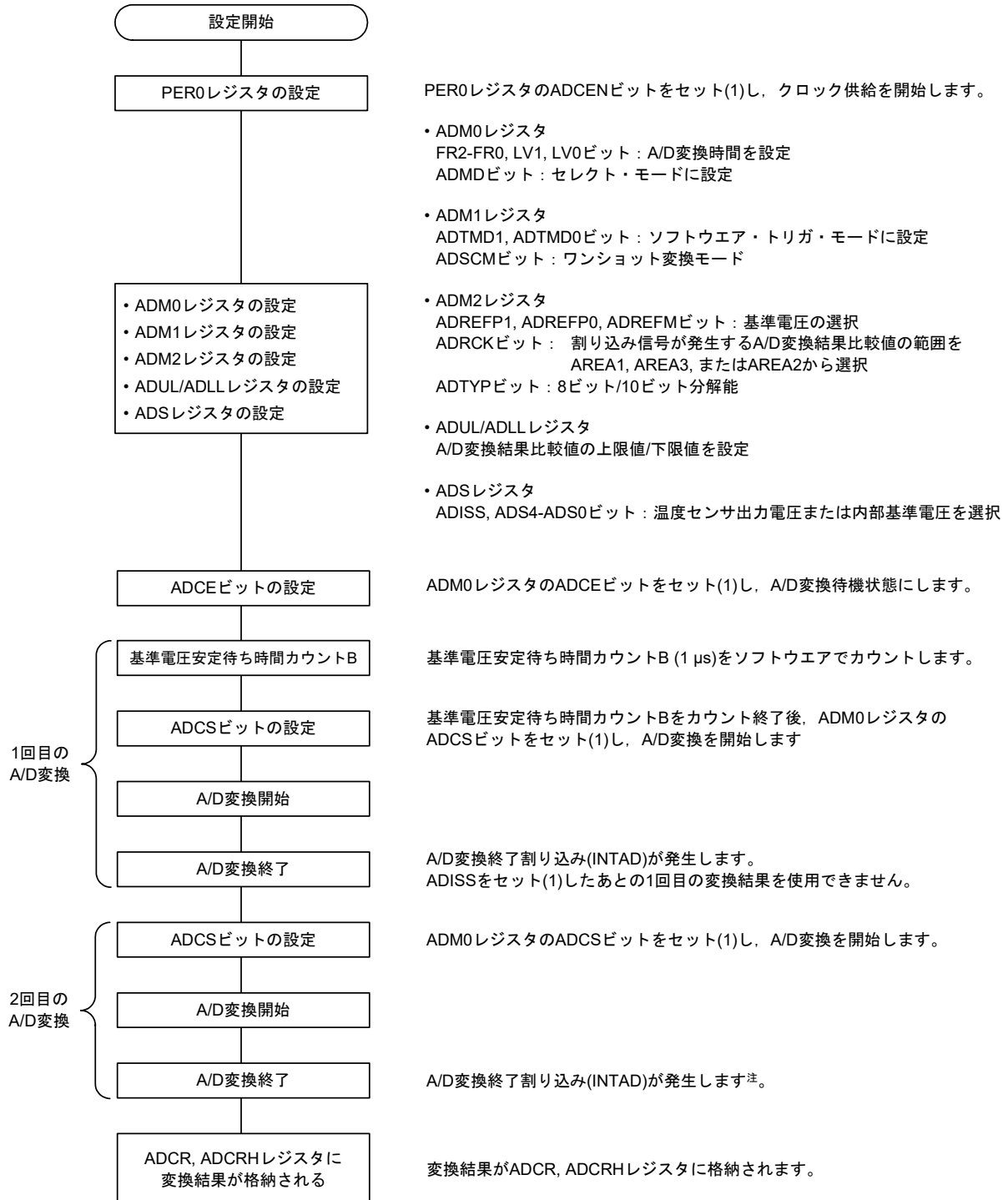
図14 - 34 温度センサ出力電圧／内部基準電圧を選択時の設定
