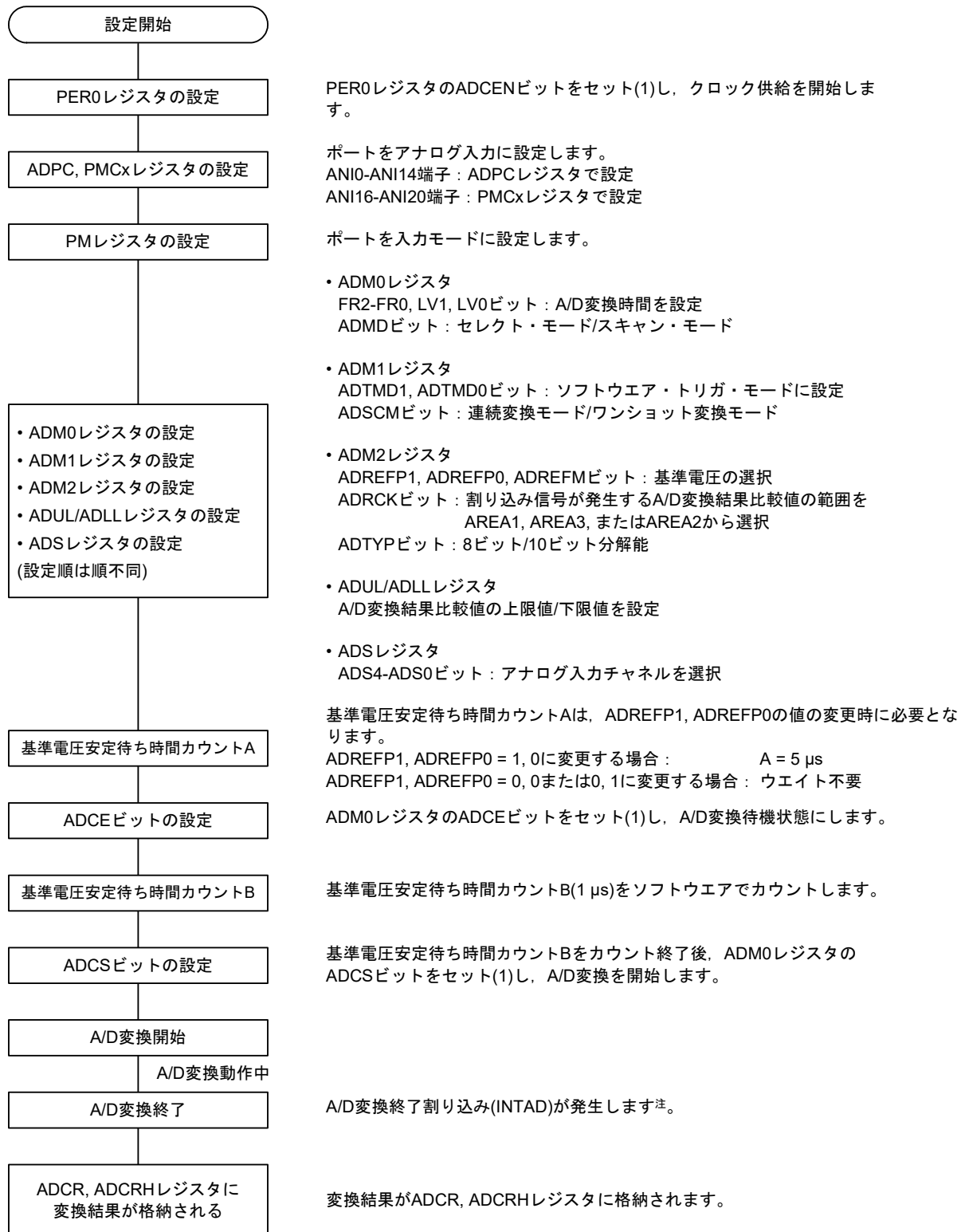
図 14 - 31 ソフトウェア・トリガ・モード設定
