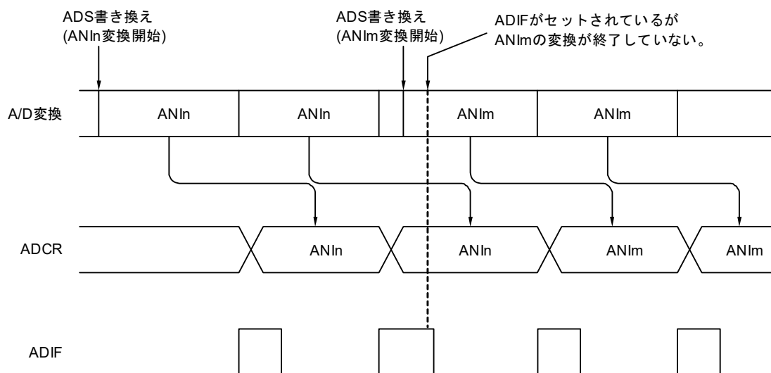
図14 - 47 A/D変換終了割り込み要求発生タイミング
