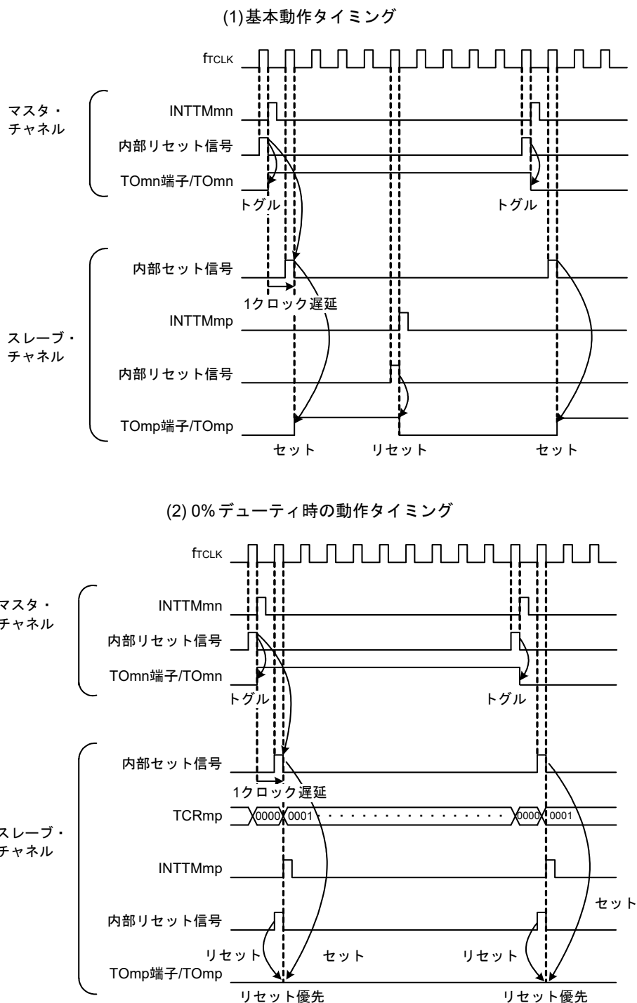
図6-40 セット/リセット・タイミング動作状態
