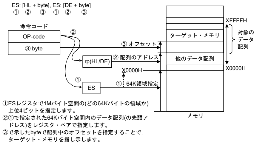
図3 - 36 ES:[HL + byte], ES:[DE + byte]の例
