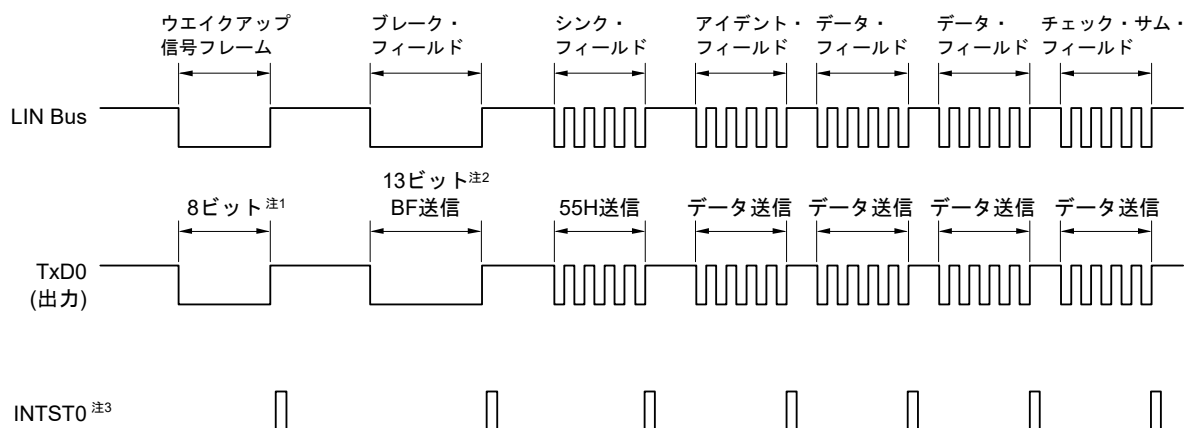
図17-131 LINの送信操作
