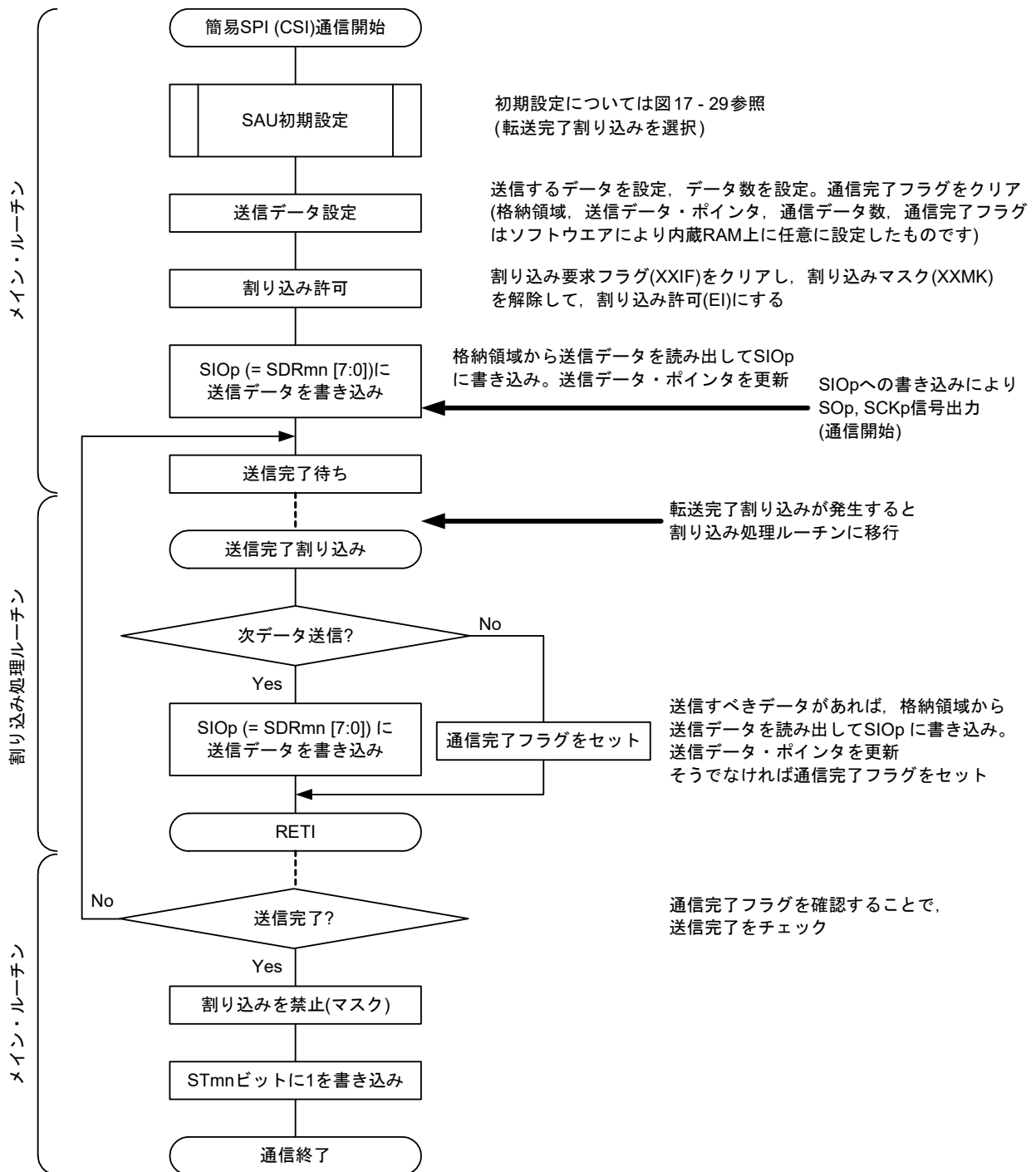
図17-33 マスタ送信(シングル送信モード時)のフロー・チャート
