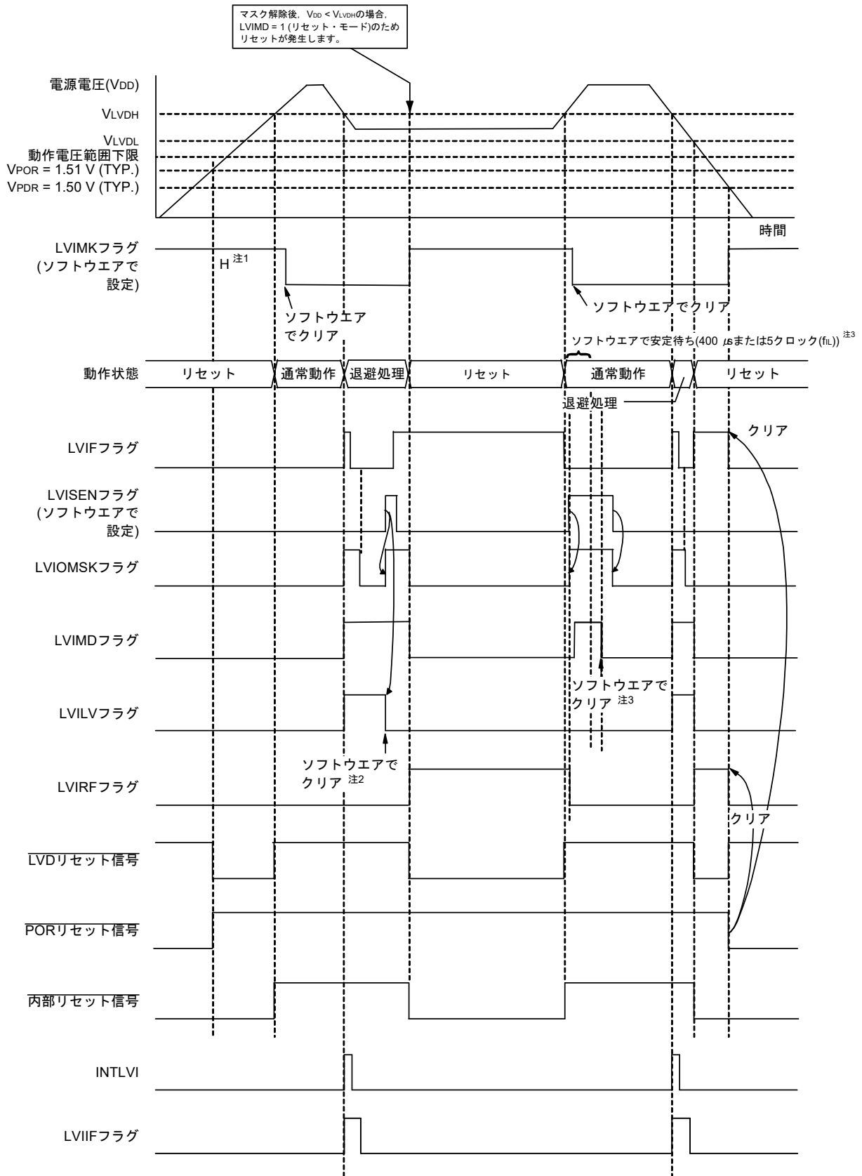
図26 - 8 割り込み&リセット信号発生タイミング(オプション・バイトLVIMDS1, LVIMDS0 = 1, 0) (2/2)
