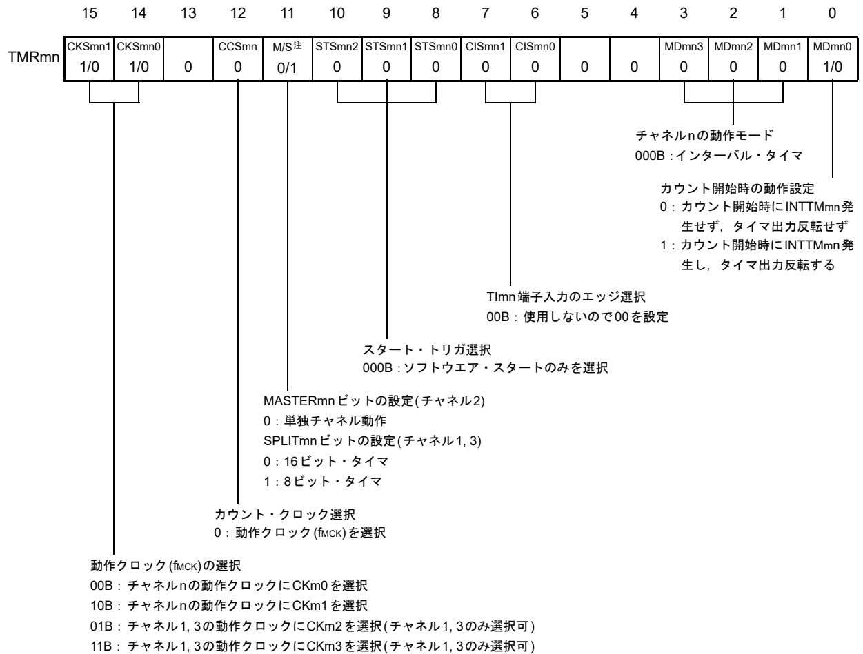
図6-48 インターバル・タイマ/方形波出力時のレジスタ設定内容例 (a) タイマ・モード・レジスタ mn (TMRmn)
