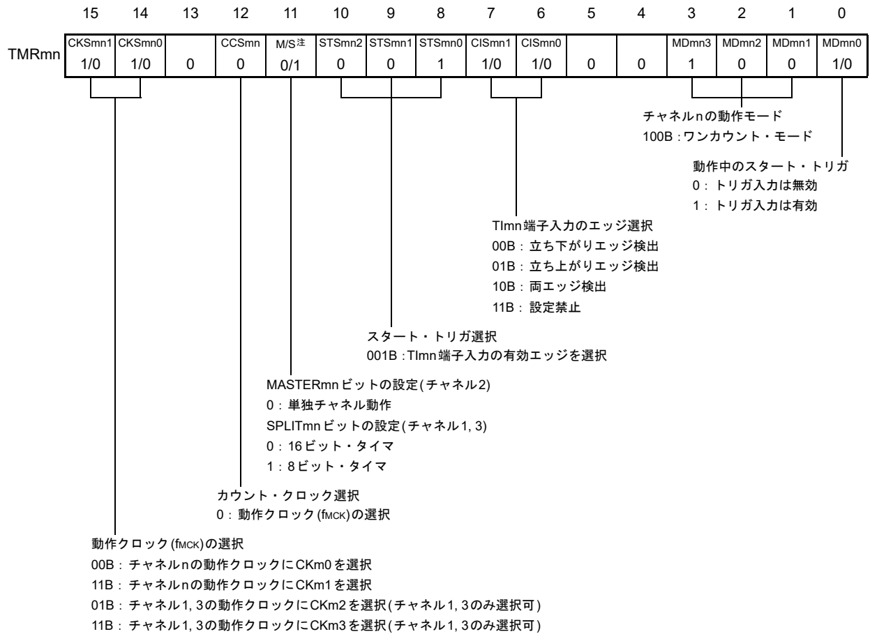
図6-69 デイレイ・カウンタ機能時のレジスタ設定内容例
