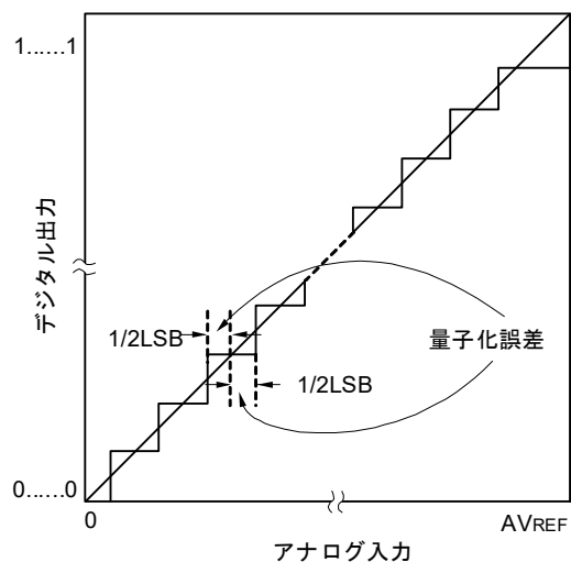
図14-41 量子化誤差
