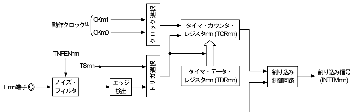
図6-67 デイレイ・カウンタとしての動作のブロック図
