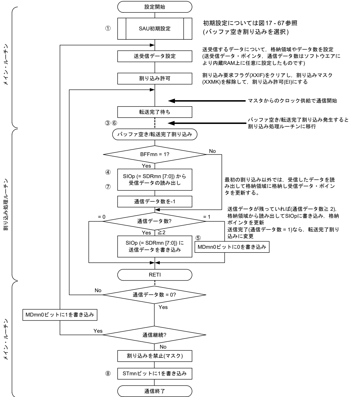
図17-73 スレーブ送受信(連続送受信モード時)のフロー・チャート
