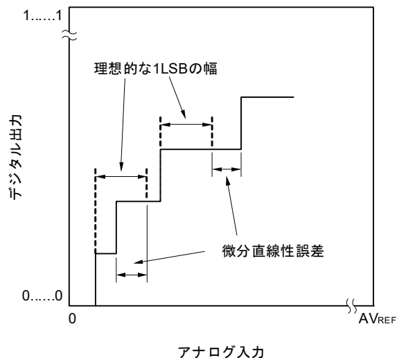
図14-45 微分直線性誤差
