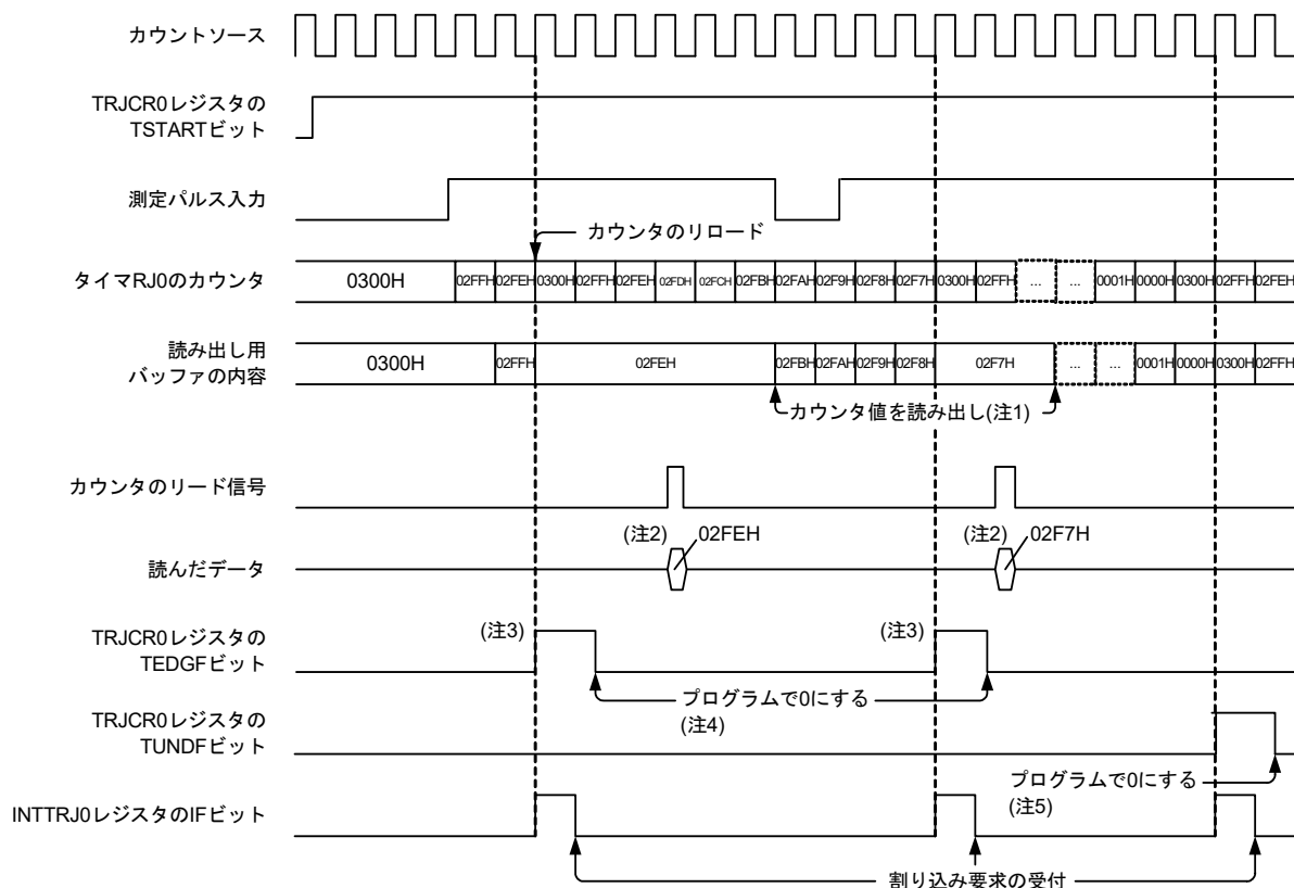
図7-16 パルス周期測定モードの動作例
