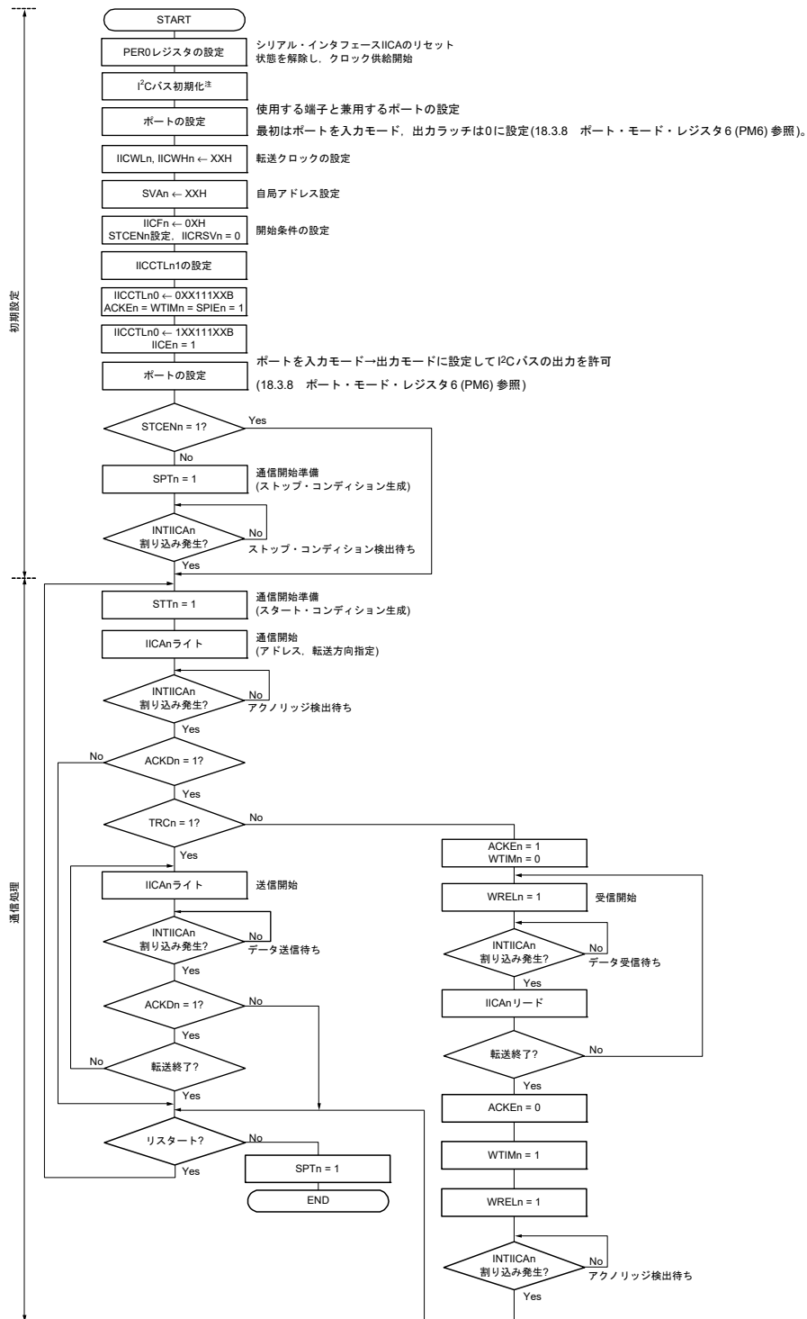
図 18 - 35 シングルマスタ・システムでのマスタ動作
