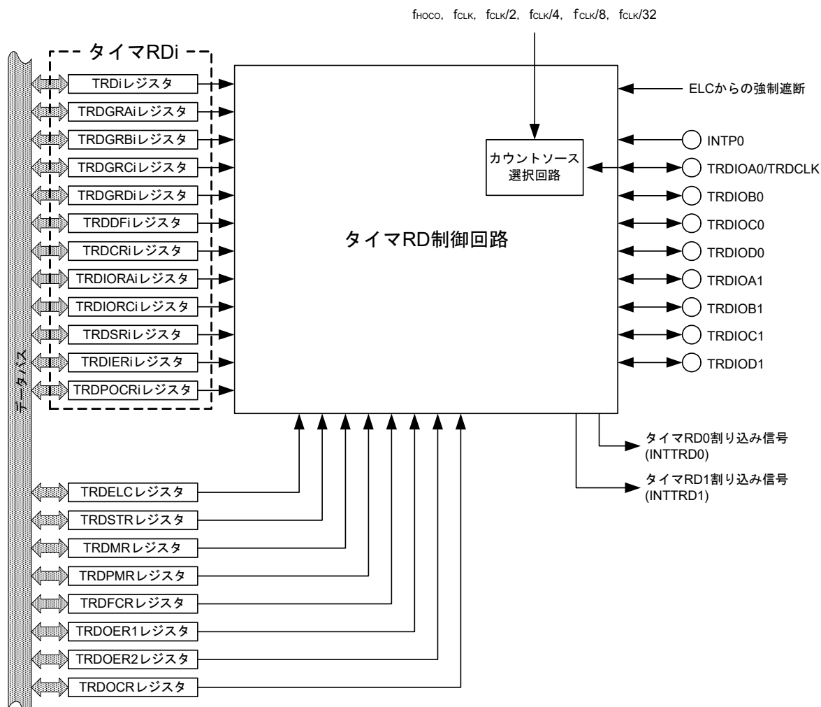
図8-1 タイマRDのブロック図
