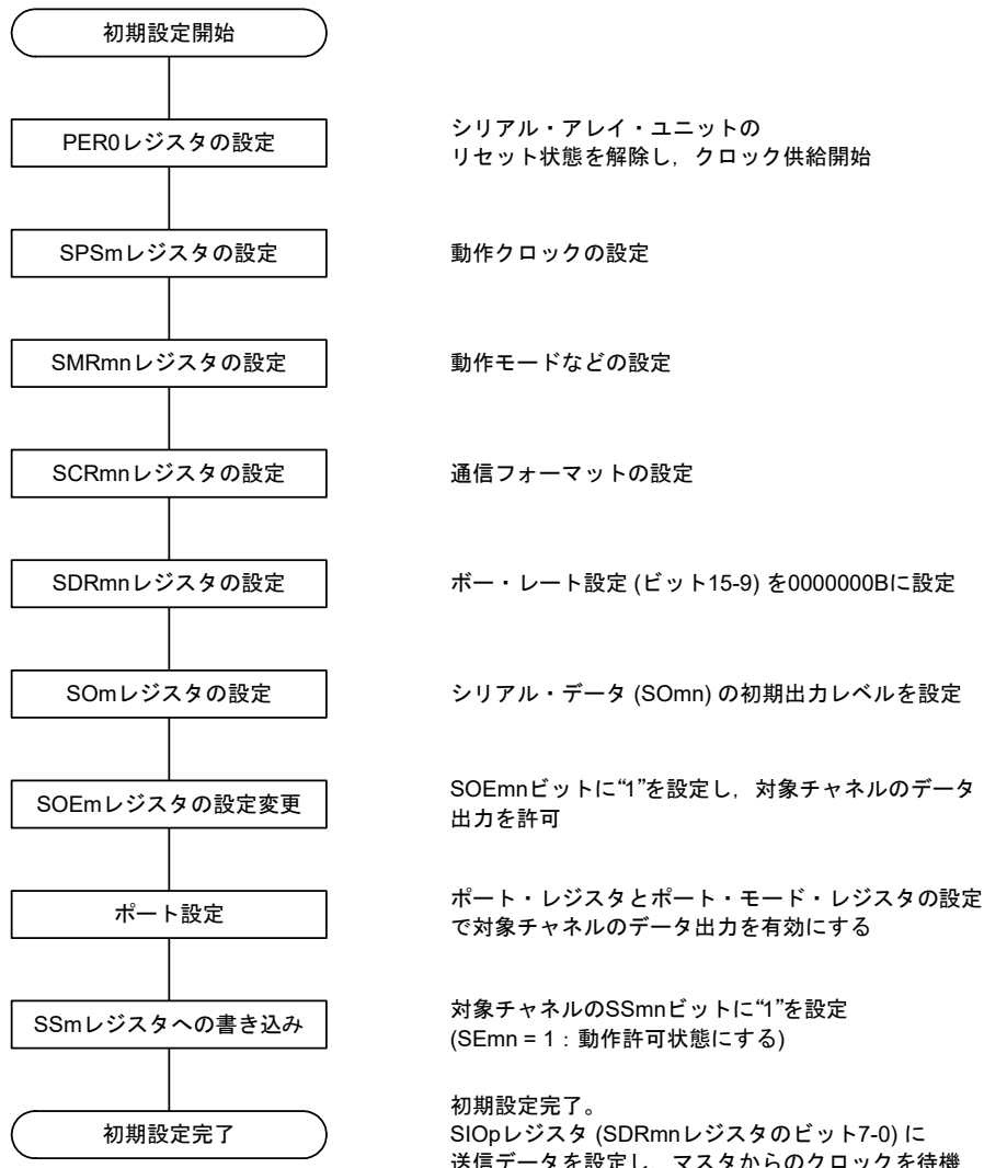
図 17 - 67 スレーブ送受信の初期設定手順
