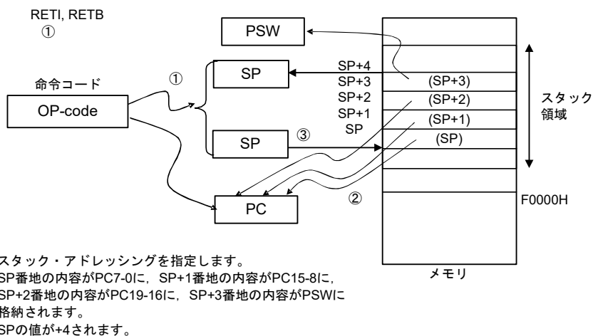
図3 - 46 RETI, RETBの例
