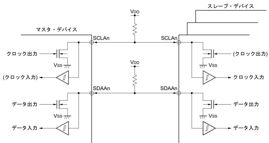
図 18 - 19 端子構成図
