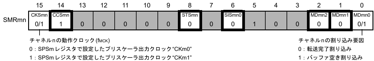
図17-97 スレーブセレクト入力機能(CSI00)のスレーブ送受信時のレジスタ設定内容例(1/2)
