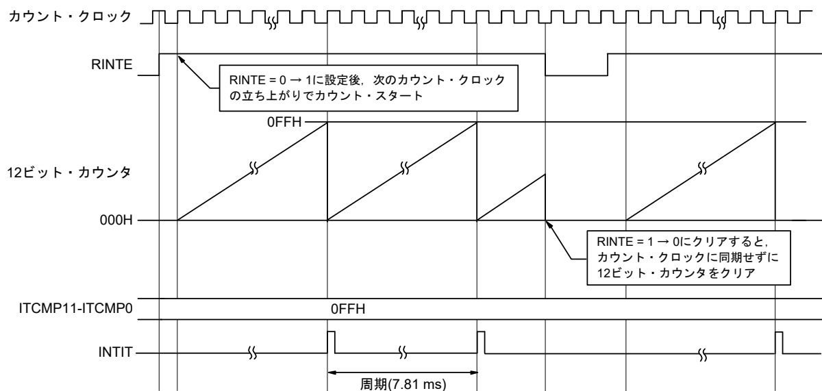
図11-5 12ビット・インターバル・タイマ動作のタイミング (ITCMP11-ITCMP0 = 0FFH, カウント・クロック : f_{SUB} = 32.768 kHz)
