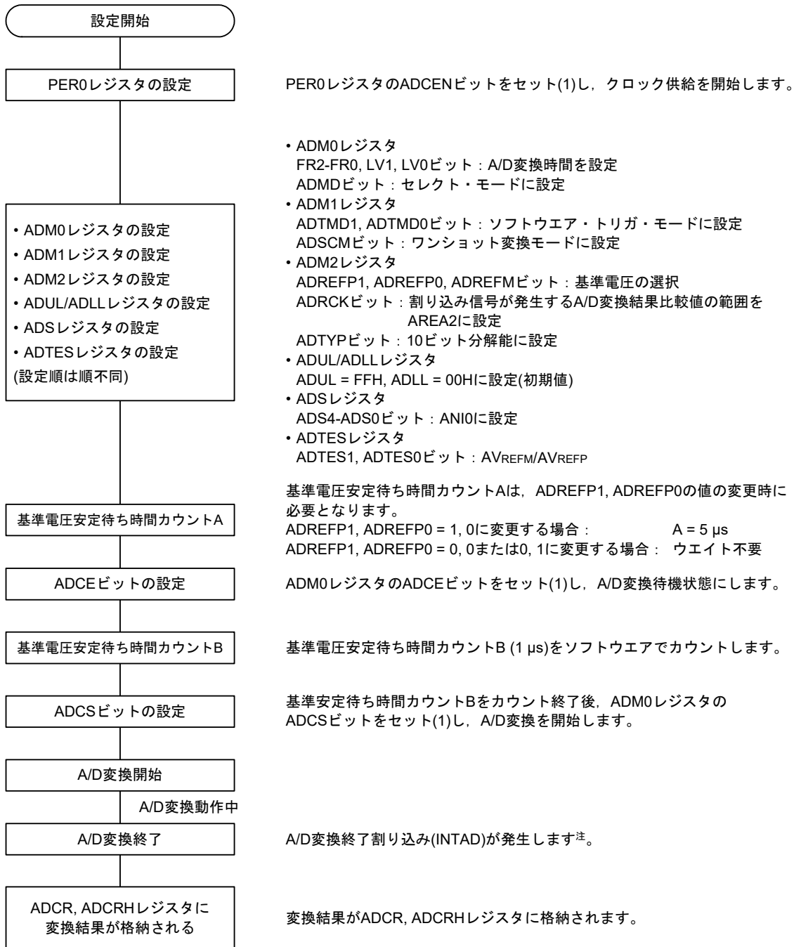
図 14 - 35 テスト・モード設定
