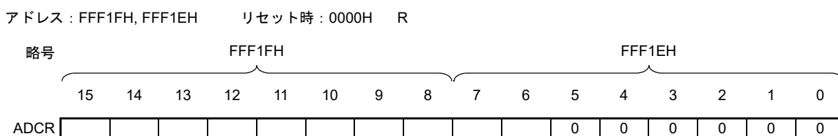
図14-10 10ビットA/D変換結果レジスタ(ADCR)のフォーマット
