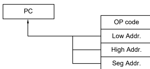
図3-20 CALL !!addr20/BR !!addr20の例
