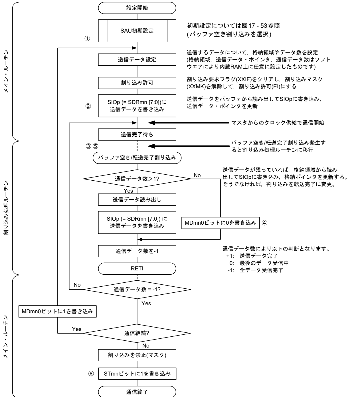
図 17 - 59 スレーブ送信(連続送信モード時)のフロー・チャート
