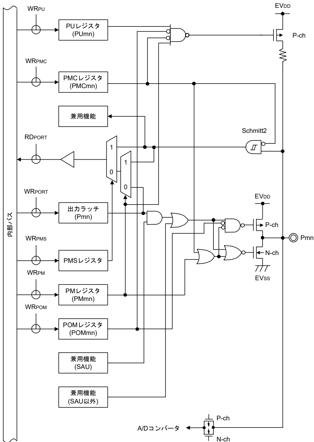
図2-12 端子タイプ7-3-4の端子ブロック図
