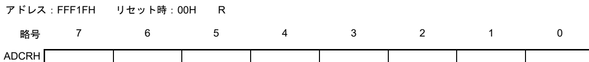
図14-11 8ビットA/D変換結果レジスタ(ADCRH)のフォーマット
