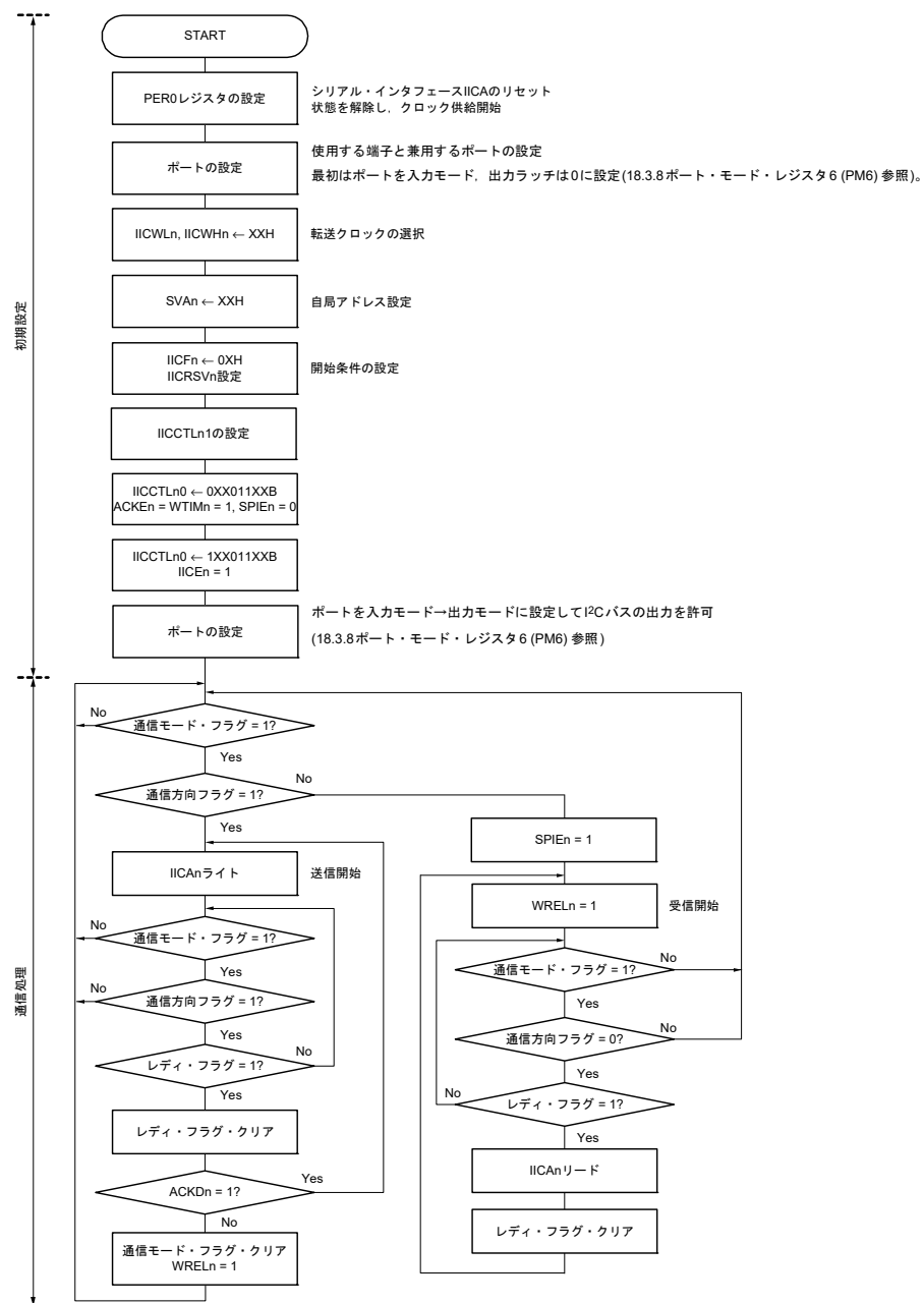
図 18 - 39 スレーブ動作手順(1)
