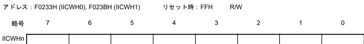
図 18 - 17 IICAハイ・レベル幅設定レジスタ n (IICWHn)のフォーマット
