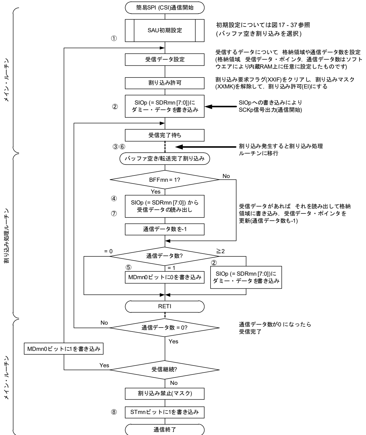
図17-43 マスタ受信(連続受信モード時)のフロー・チャート
