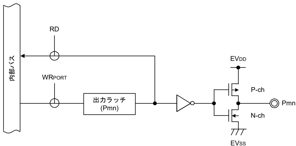
図2-1 端子タイプ 1-1-1 の端子ブロック図
