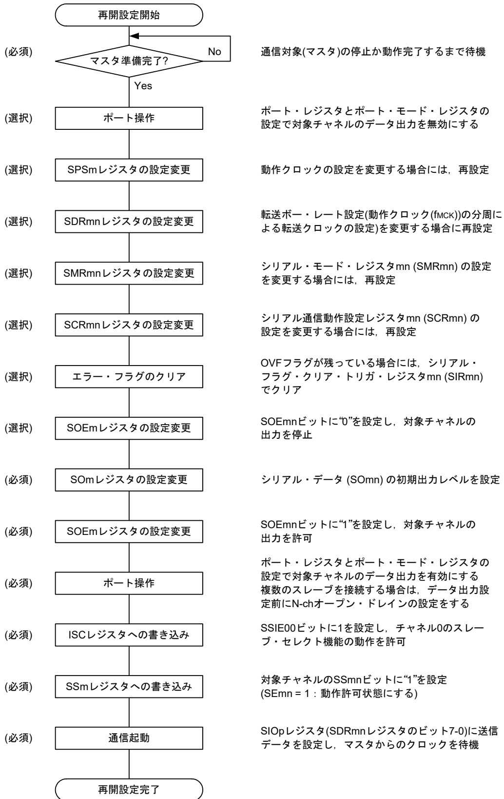
図 17 - 85 スレーブ送信の再開設定手順
