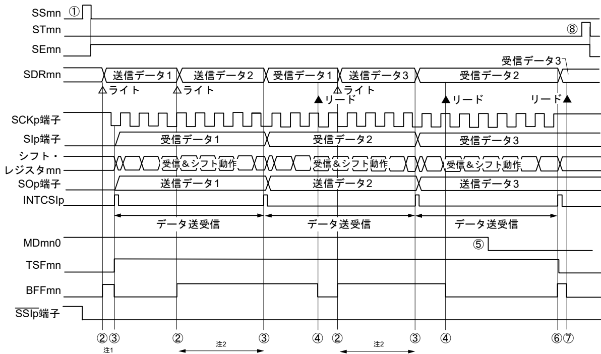
図17 - 104 スレーブ送受信 (連続送受信モード時)のタイミング・チャート (タイプ1 : DAPmn = 0, CKPmn = 0)
