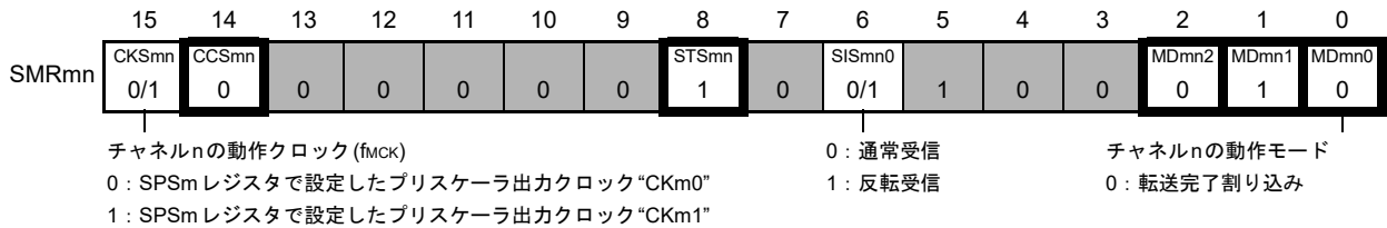
図17 - 116 UART (UART0-UART3)のUART受信時のレジスタ設定内容例(1/2)
