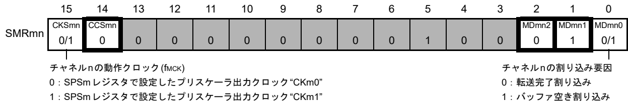
図17 - 107 UART (UART0-UART3)のUART送信時のレジスタ設定内容例(1/2)
