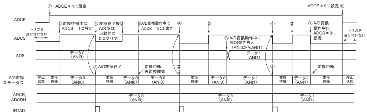
図14-20 ソフトウェア・セレクト・モード(セレクト・モード, ワンショット変換モード)動作タイミング例
