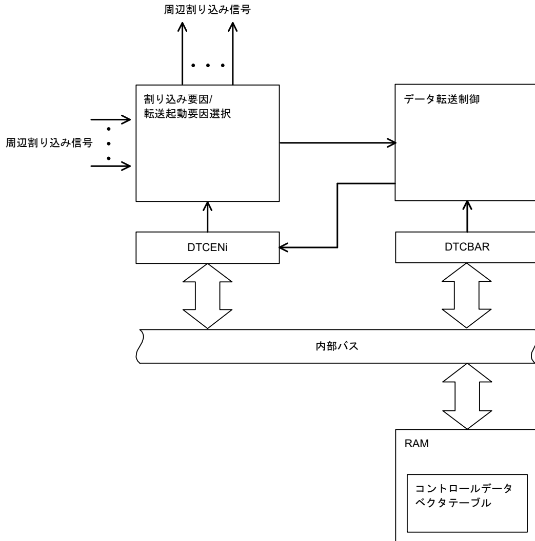
図19-1 DTCのブロック図
