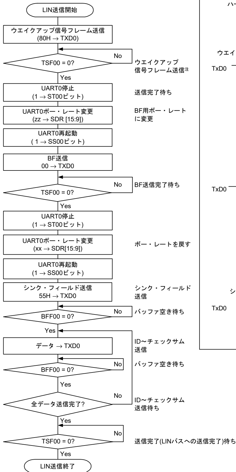
図 17 - 132 LIN送信のフロー・チャート
