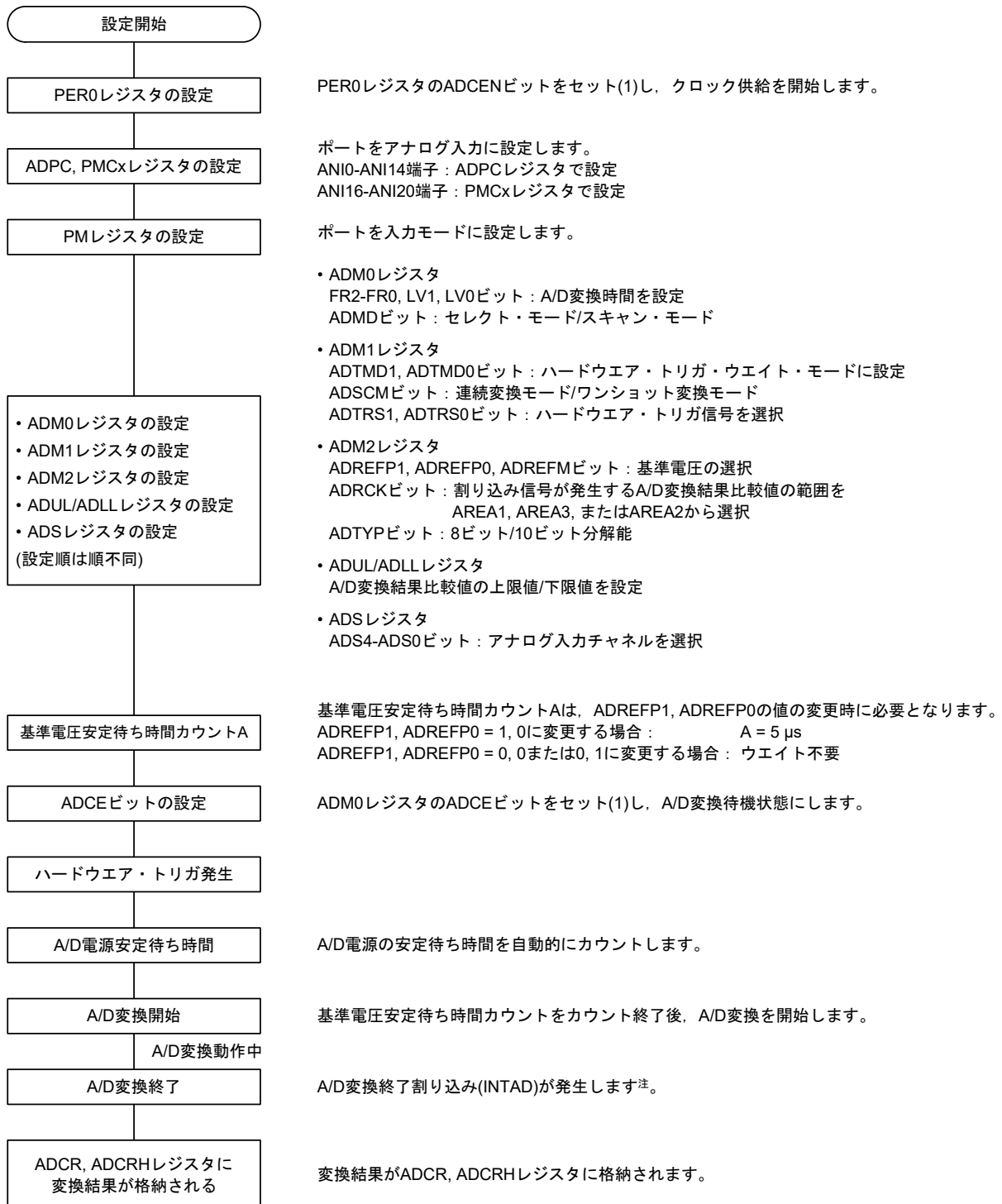
図14-33 ハードウェア・トリガ・ウェイト・モード設定
