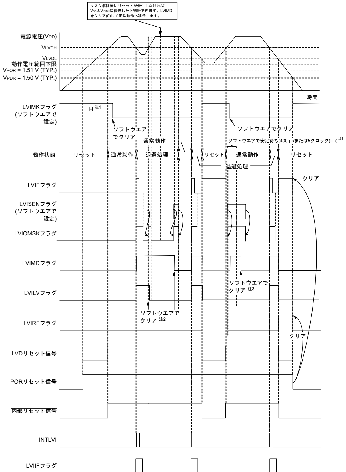
図26 - 7 割り込み&リセット信号発生タイミング(オプション・バイトLVIMDS1, LVIMDS0 = 1, 0) (1/2)
