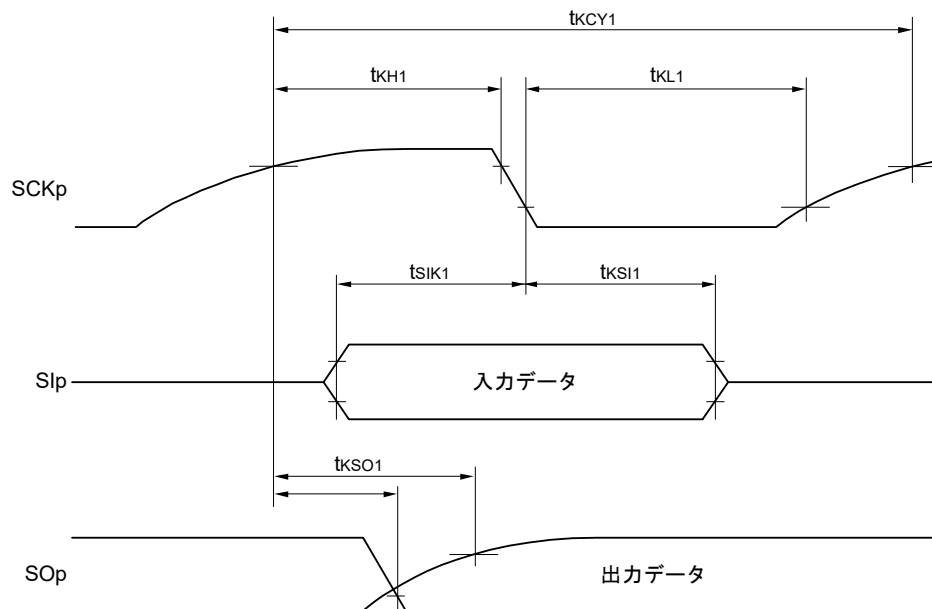
簡易SPI (CSI)モード・シリアル転送タイミング：マスタ・モード(異電位通信時) (DAPmn = 0, CKPmn = 1またはDAPmn = 1, CKPmn = 0のとき)
