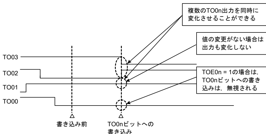
図6 - 42 TO0nビットの一括操作によるTO0nの端子状態
