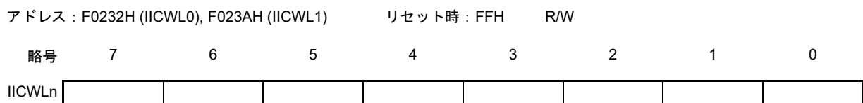
図 18 - 16 IICAロウ・レベル幅設定レジスタ n (IICWLn)のフォーマット
