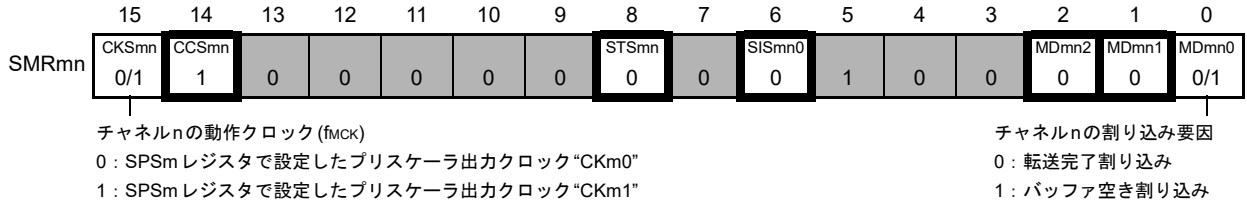
図 17 - 81 スレーブセレクト入力機能(CSI00)のスレーブ送信時のレジスタ設定内容例(1/2)
