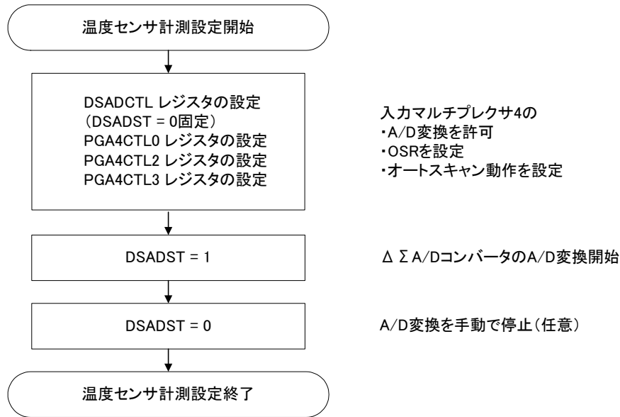
図14-42 プログラマブル・ゲイン計装アンプ付き24ビット \Delta\Sigma /Dコンバータの温度センサ計測フロー
