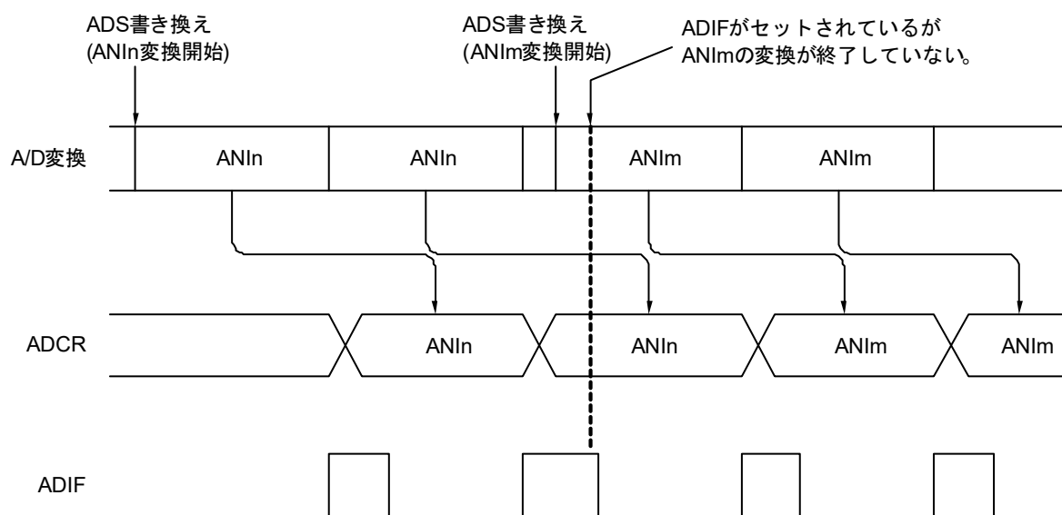
図16-47 A/D変換終了割り込み要求発生タイミング
