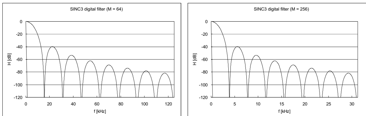
図14-38 SINC3フィルタの周波数応答
