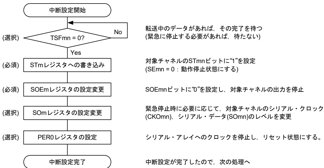
図 19 - 44 マスタ送受信の中断手順
