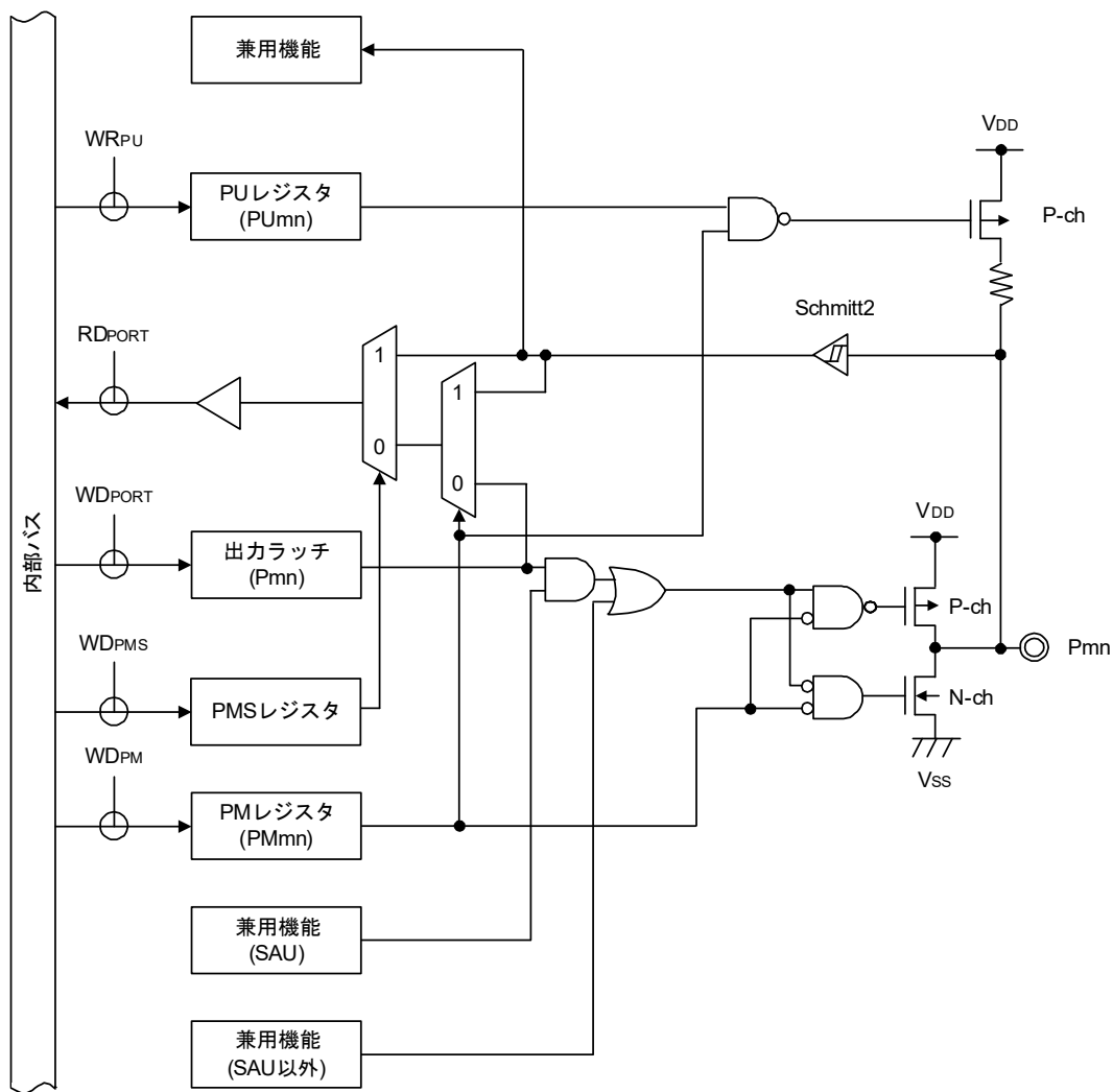
図2-4 端子タイプ7-1-3の端子ブロック図
