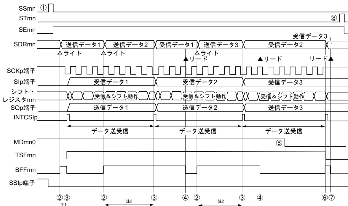
図19 - 102 スレーブ送受信 (連続送受信モード時)のタイミング・チャート (タイプ1 : DAPmn = 0, CKPmn = 0)
