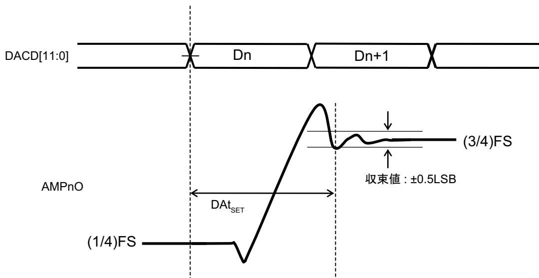
図18-7 12ビットD/Aコンバータの動作例
