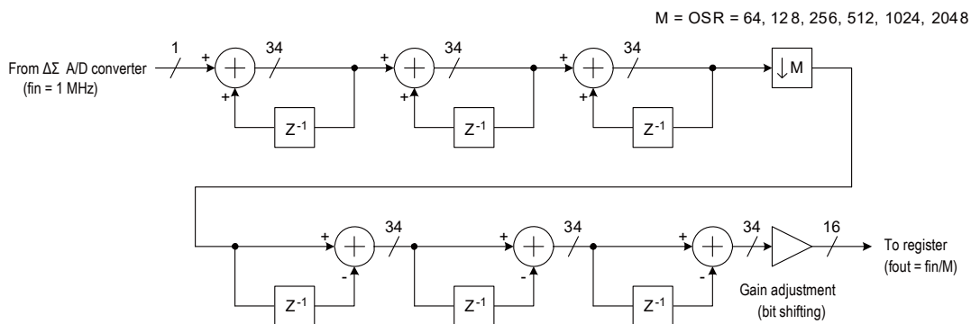
図14-37 デジタル・フィルタのブロック図
