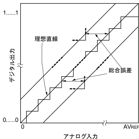
図 16 - 40 総合誤差
