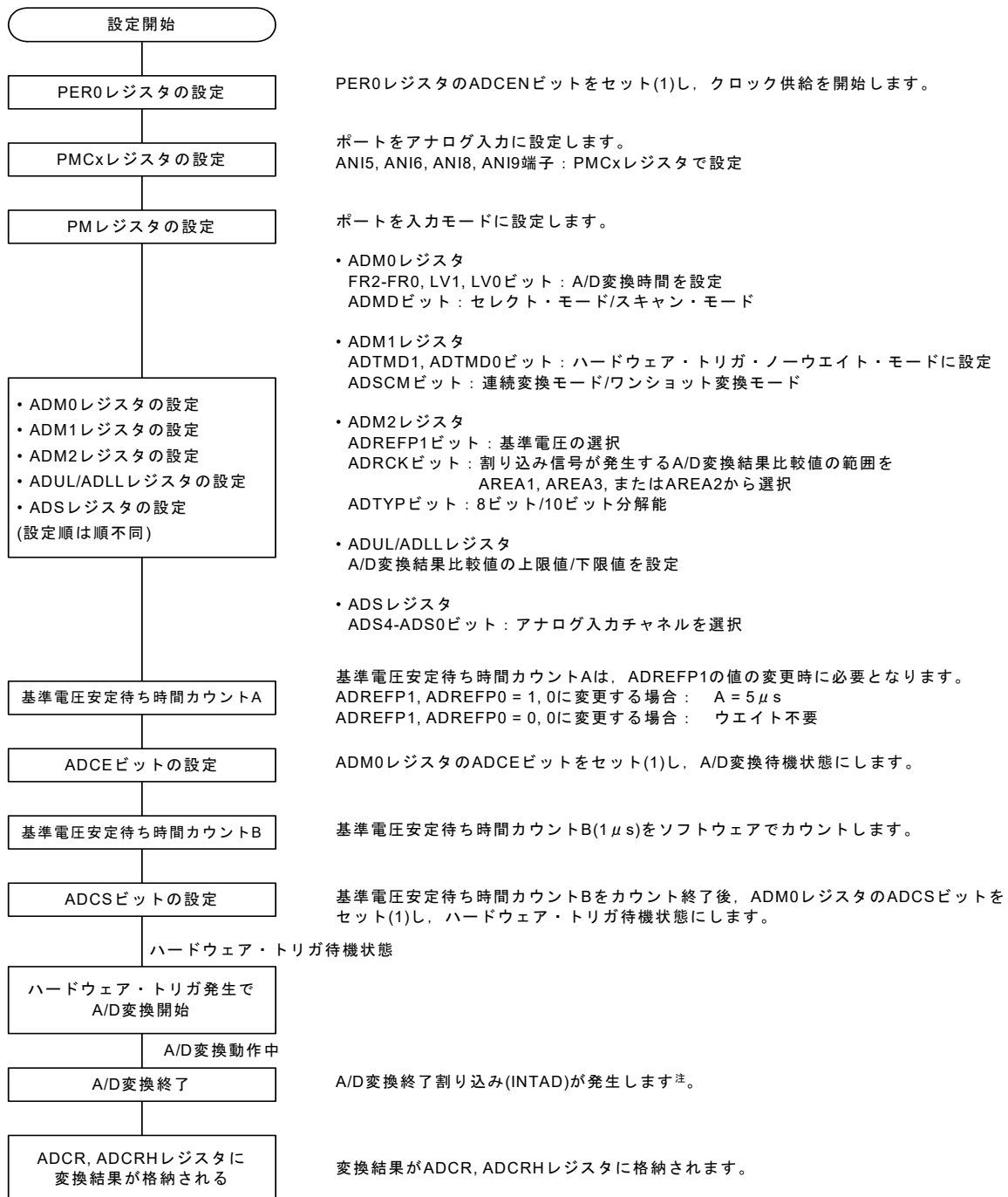
図16-32 ハードウェア・トリガ・ノーウエイト・モード設定
