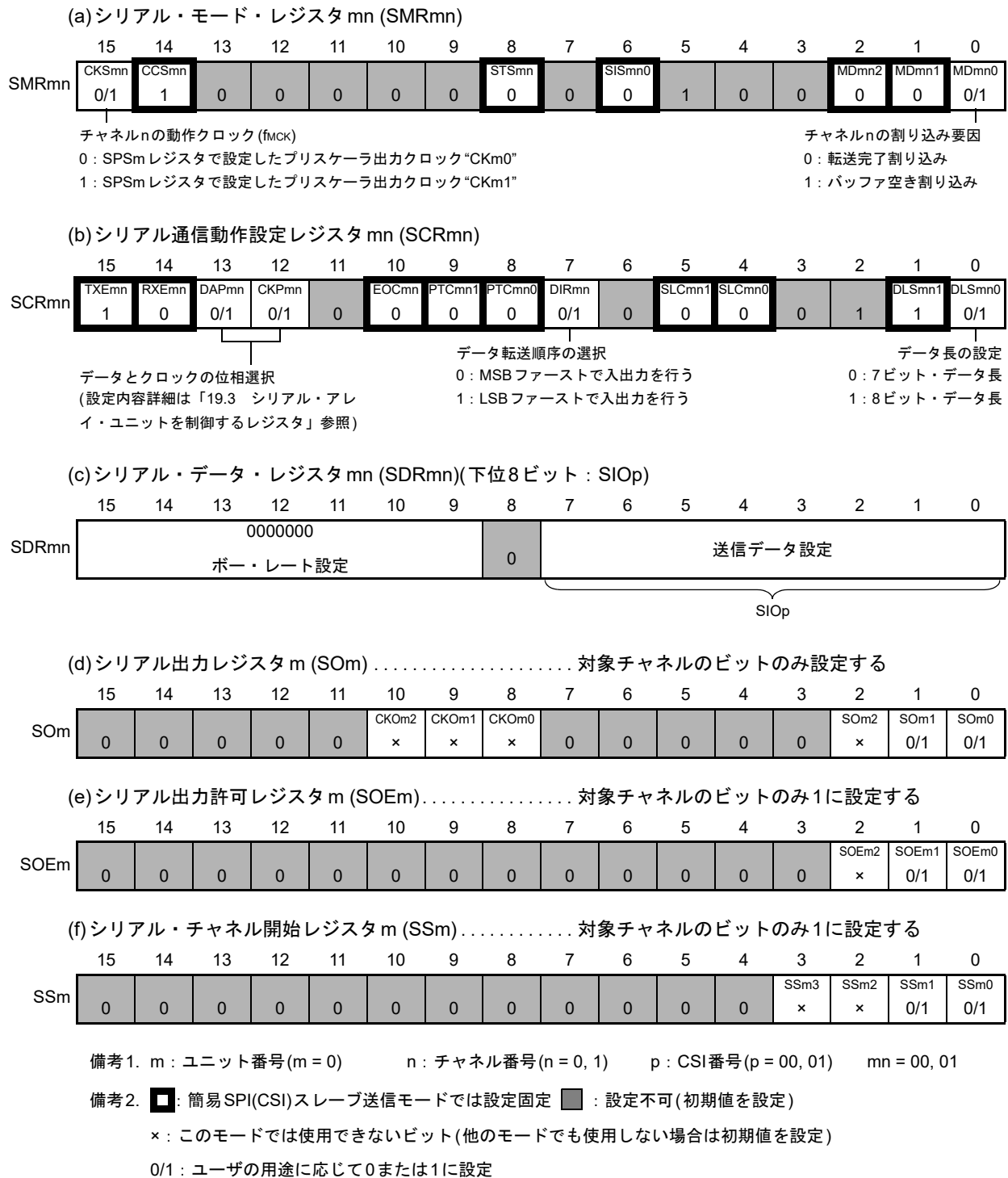
図19 - 50 簡易SPI (CSI00, CSI01)のスレーブ送信時のレジスタ設定内容例
