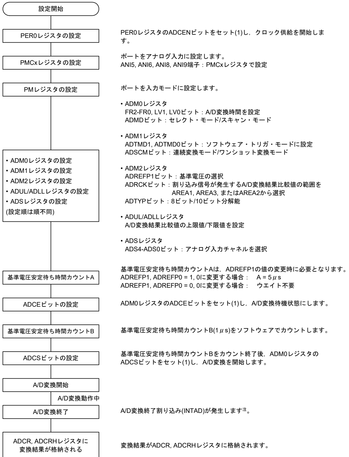
図16-31 ソフトウェア・トリガ・モード設定
