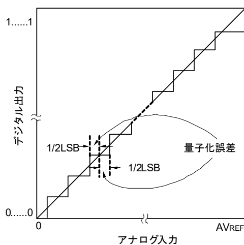
図 16 - 41 量子化誤差
