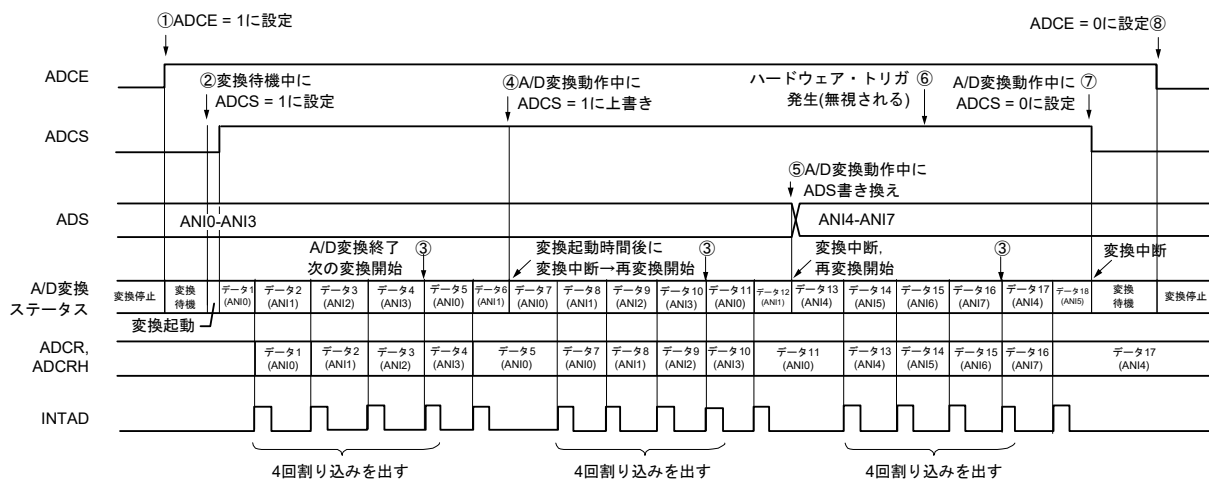
図16-21 ソフトウェア・トリガ・モード(スキャン・モード, 連続変換モード)動作タイミング例
