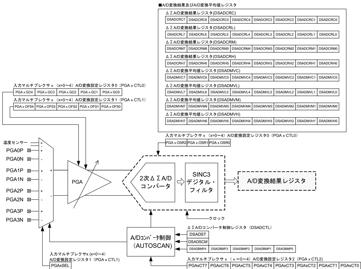
図14-12 24ビット \Delta\Sigma A/Dコンバータのブロック図
