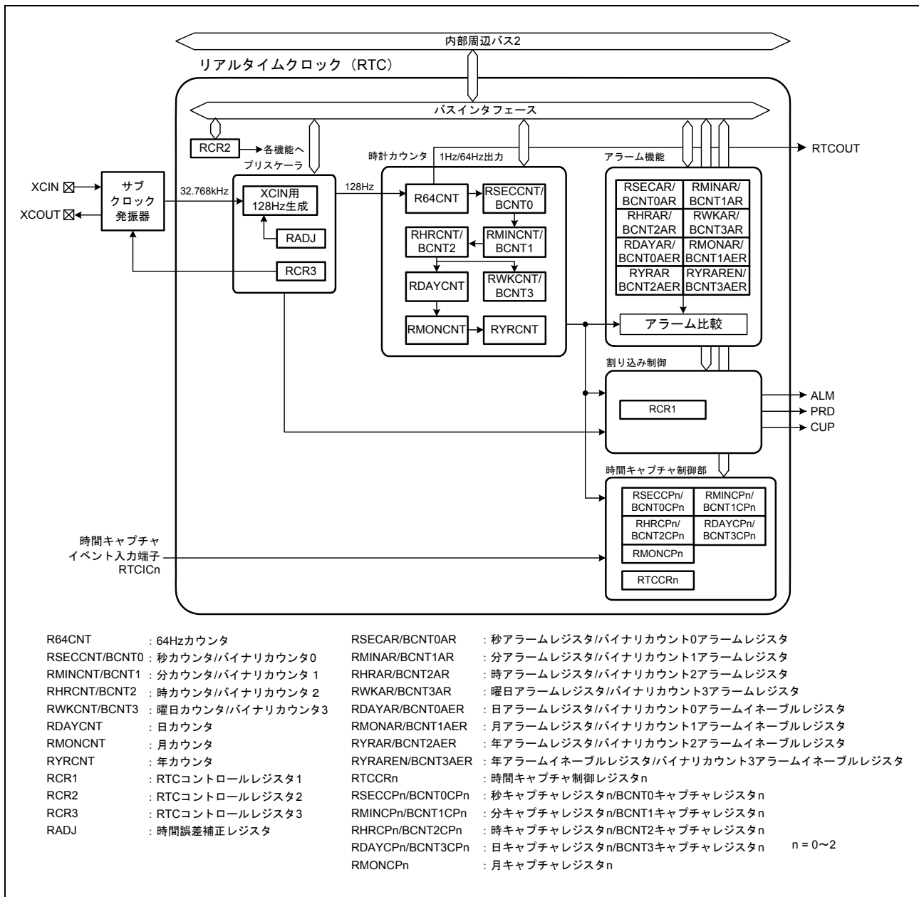
図 26.1 RTCのブロック図
