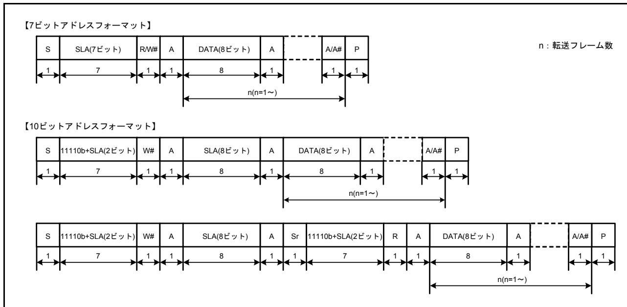
図 31.3 I 2 C バスフォーマット
