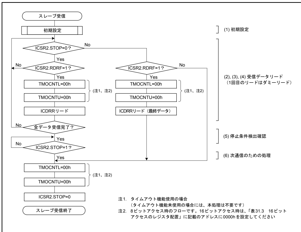
図 31.18 スレーブ受信のフローチャート例
