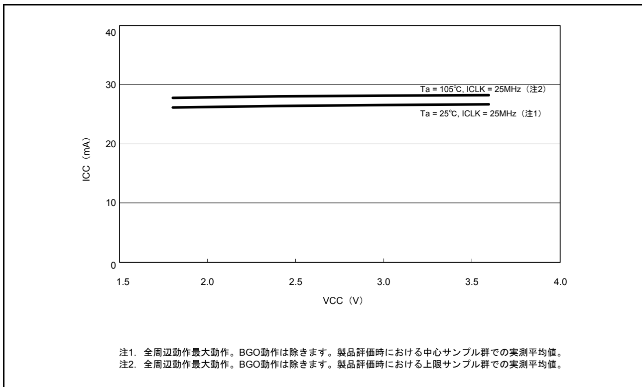
図 44.2 中速動作モード 1A、1B の電圧依存性（参考データ）
