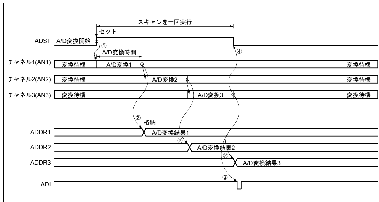
図 35.3 シングルスキャンモードの動作例 (基本動作)
