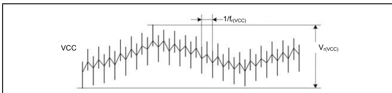
図 44.10 電源リップル波形
