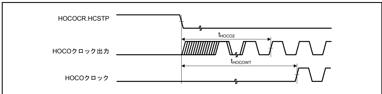
図 44.29 HOCO クロック発振開始タイミング (HOCOCR.HCSTP ビット設定による発振開始)
