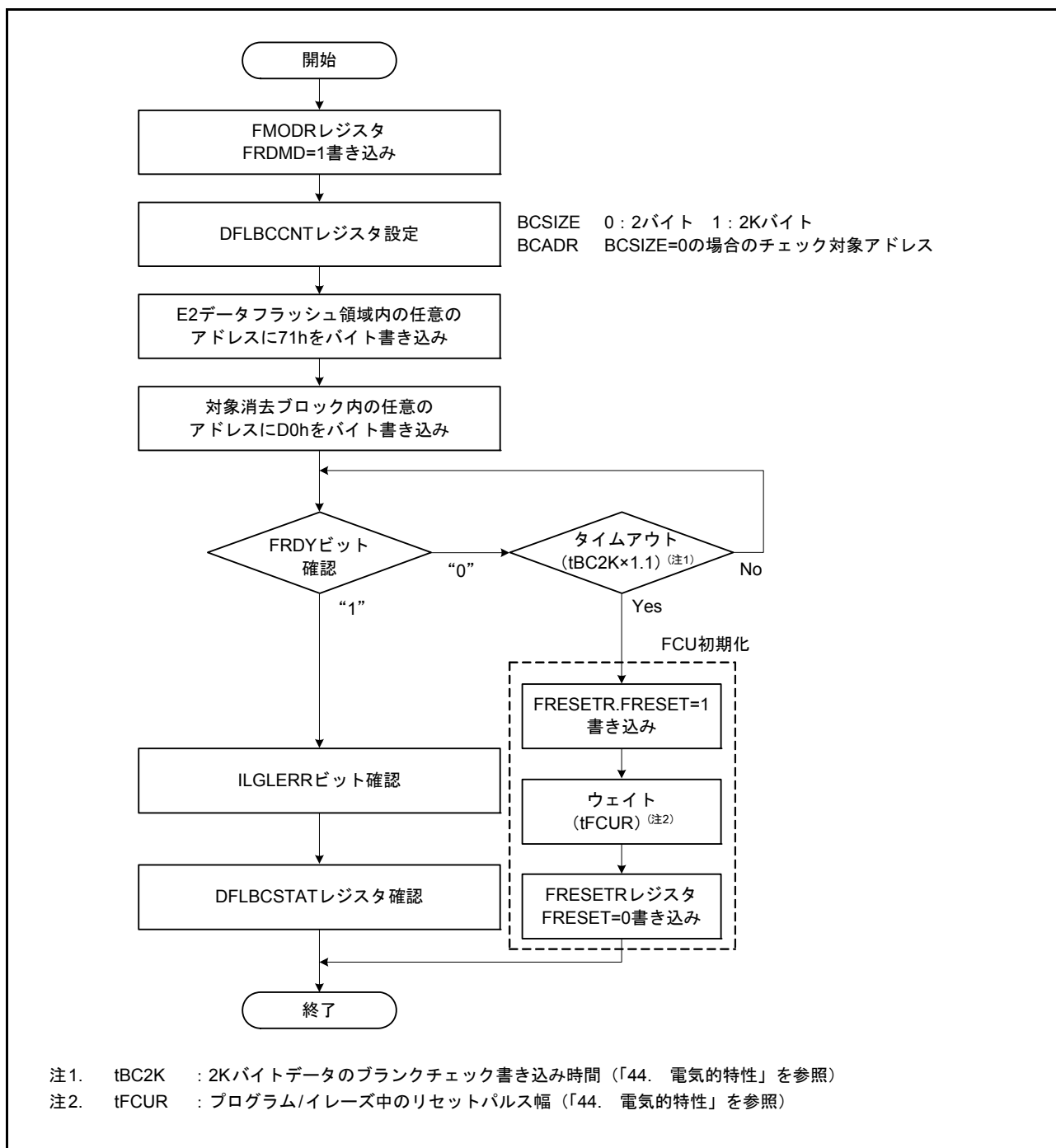
図 43.6 E2 データフラッシュのブランクチェック
