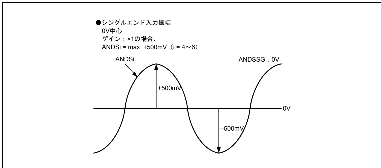
図 44.56 シングルエンド入力振幅
