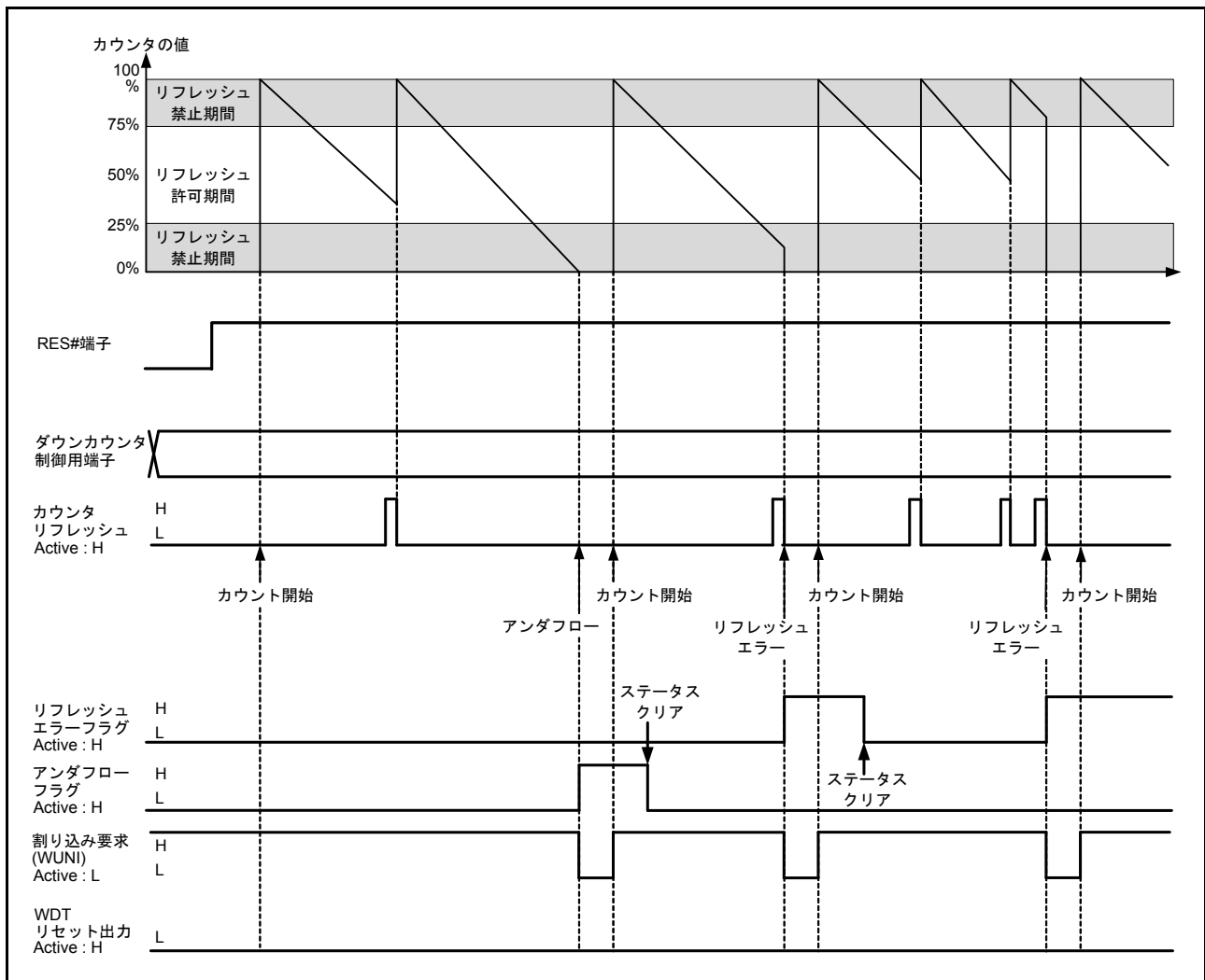
図 27.4 オートスタートモード動作例
