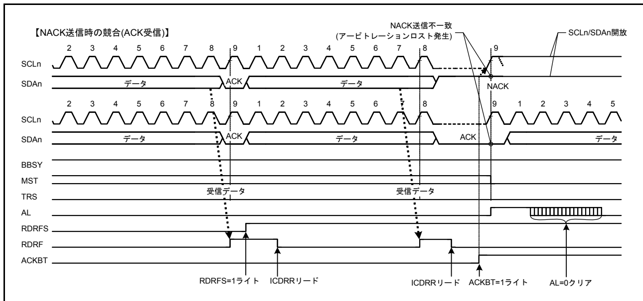
図 31.35 NACK 送信アービトレーションロスト検出動作例 (NALE=1 のとき)
