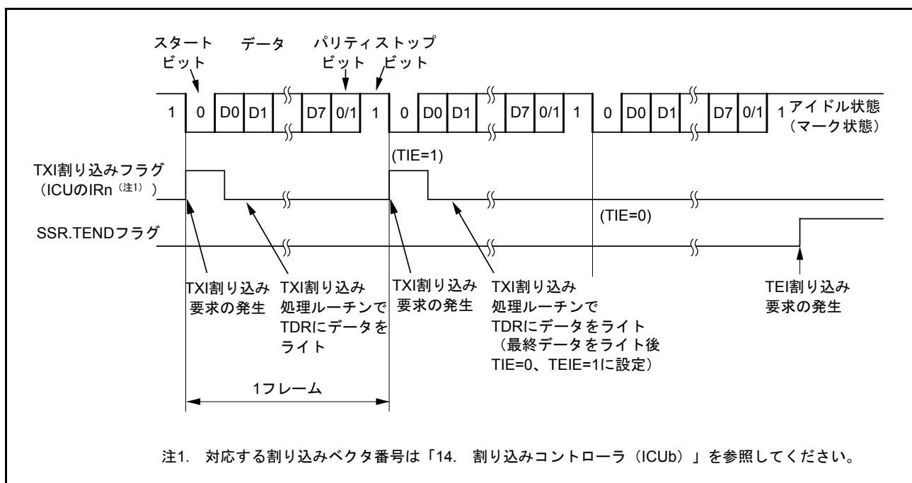
図 29.8 調歩同期式モードのシリアル送信（送信中～送信終了時）の動作例（8 ビットデータ / パリティあり / 1 ストップビットの例）
