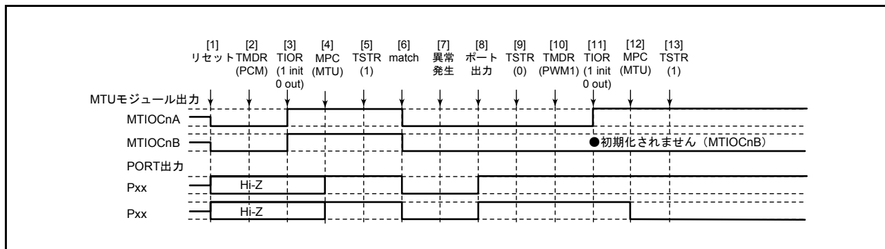
図 22.142 位相計数モードで異常が発生し、PWM モード1で復帰する場合
