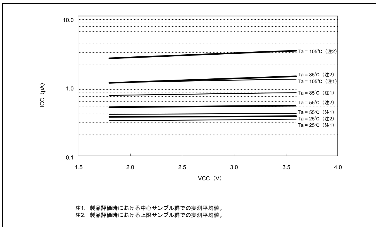
図 44.8 ディープソフトウェアスタンバイモード (DEEPCUT1 ビット = 1) 時の電圧依存性 (参考データ)
