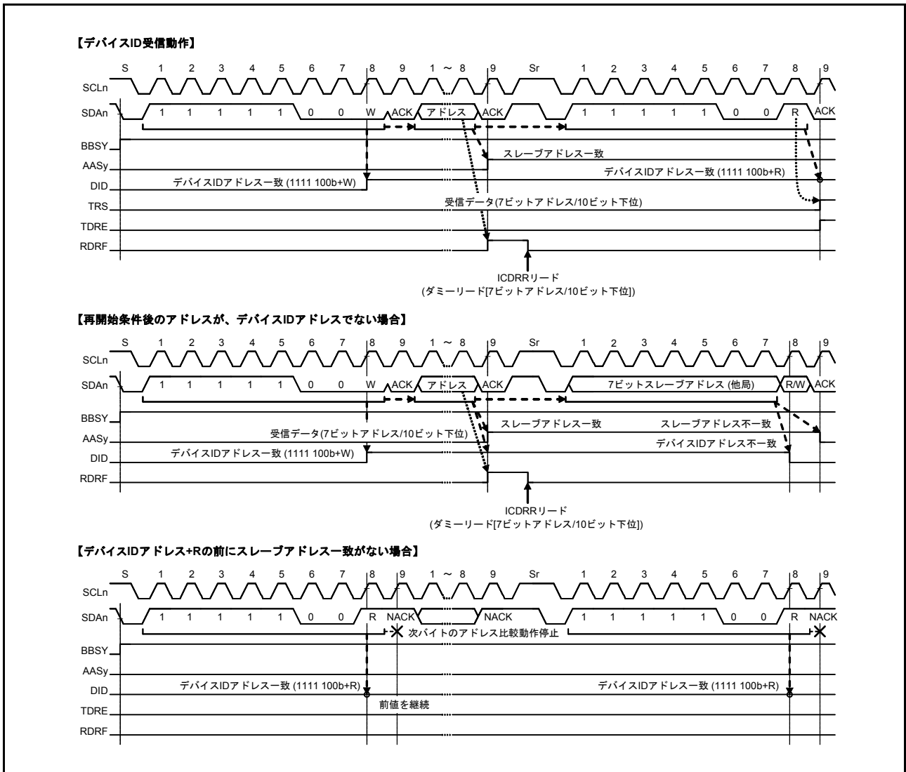
図 31.28 デバイス ID アドレス受信時の AASy、DID フラグセット/クリアタイミング
