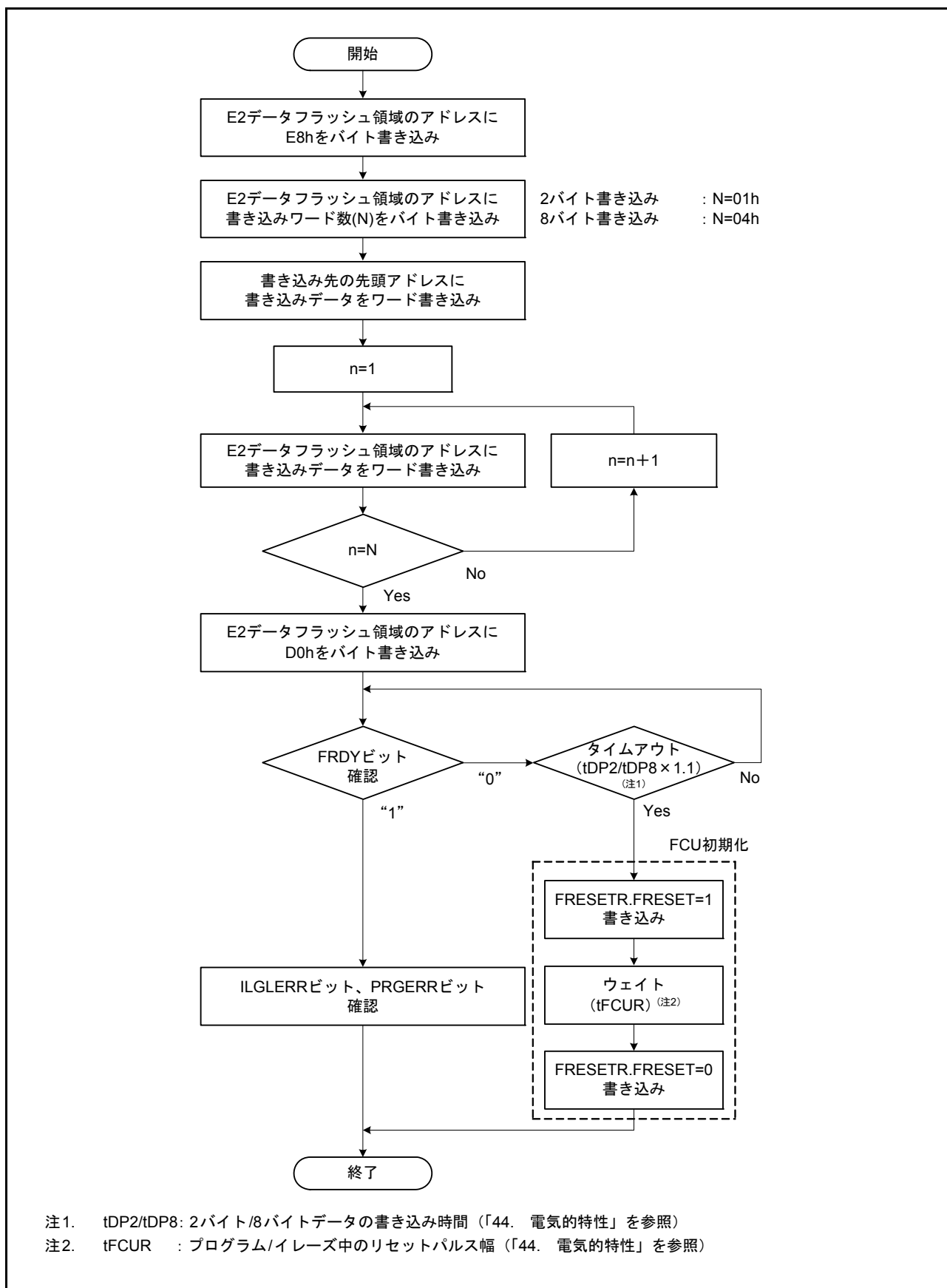
図 43.5 E2 データフラッシュの書き込み
