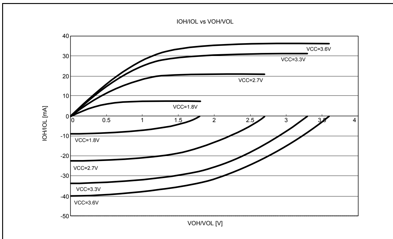
図 44.16 高駆動出力を選択したときの VOH/VOL、IOH/IOL 電圧特性 Ta = 25 °C (参考データ)
