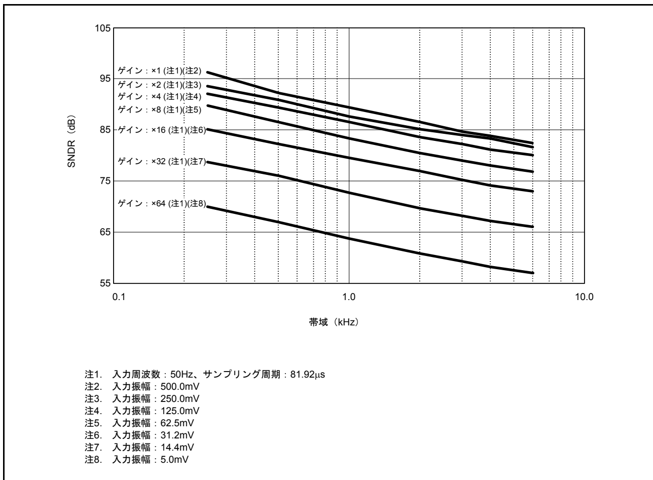
図 44.60 SNDR の帯域依存性 (参考データ)
