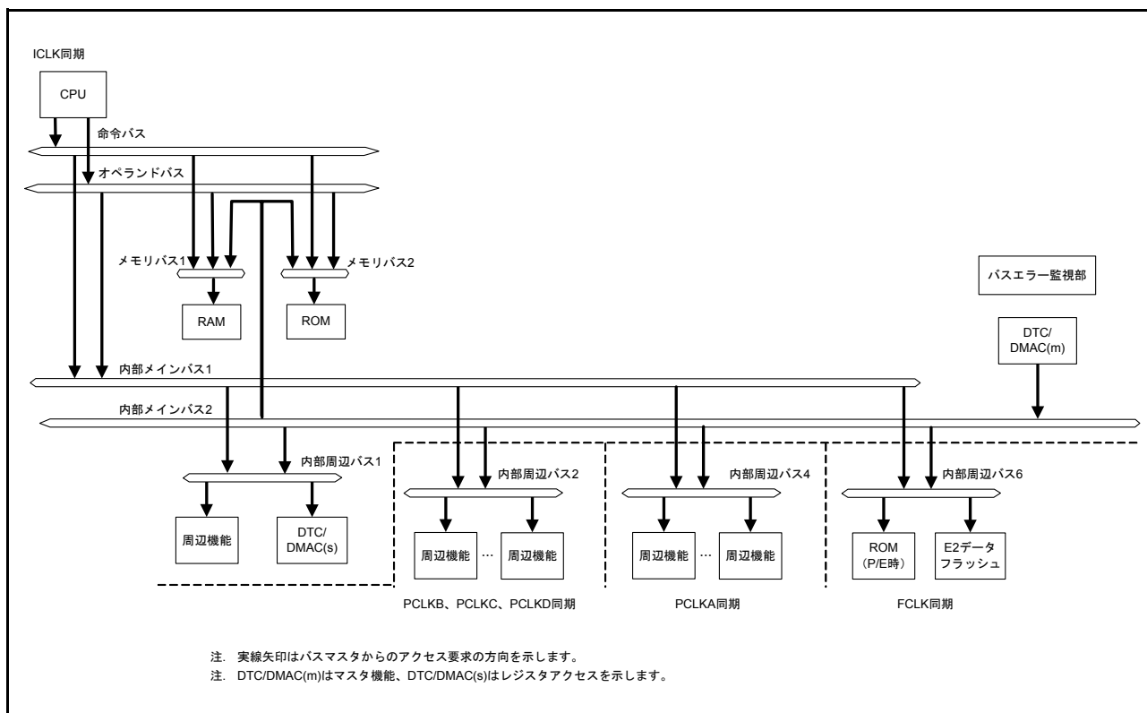
図 15.1 バスの構成図
