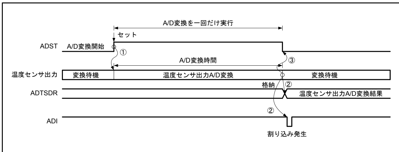
図 35.5 シングルスキャンモードの動作例 (温度センサ出力選択)
