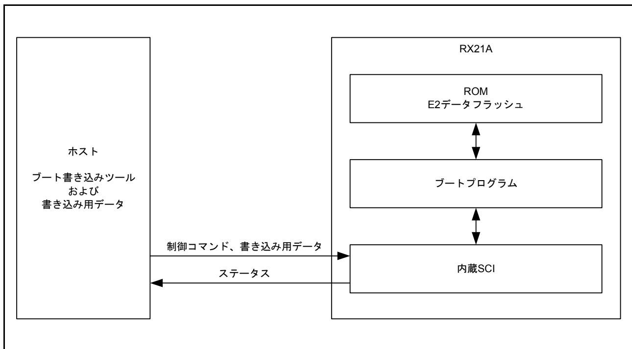
図 42.21 ブートモード時のシステム構成
