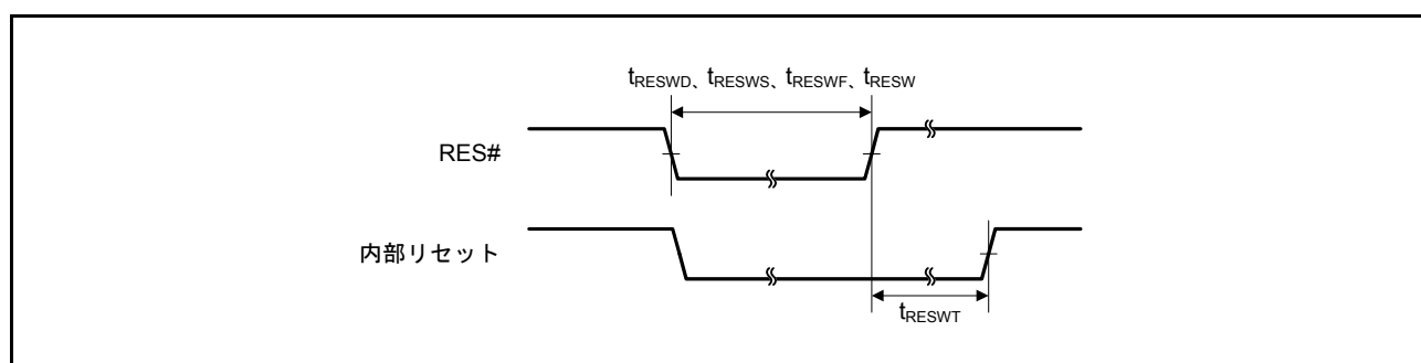
図 44.36 リセット入力タイミング
