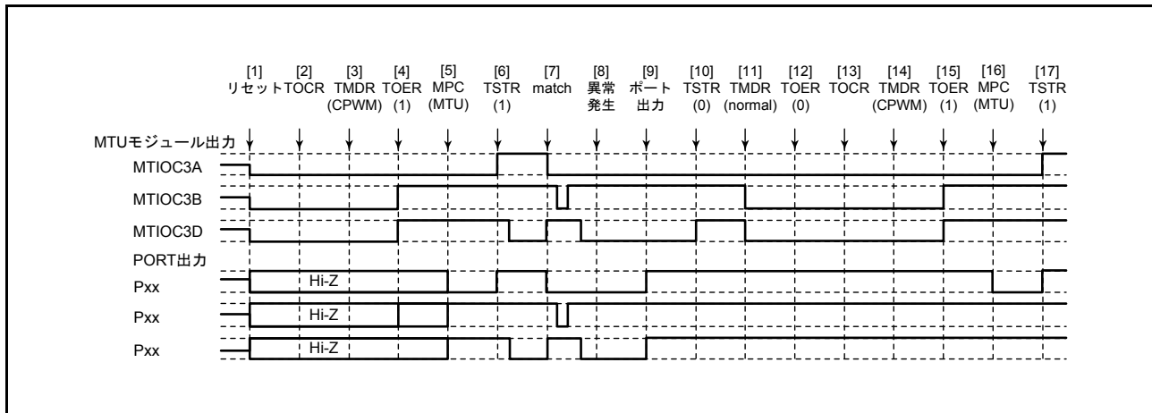
図 22.148 相補 PWM モードで異常が発生し、相補 PWM モードで復帰する場合
