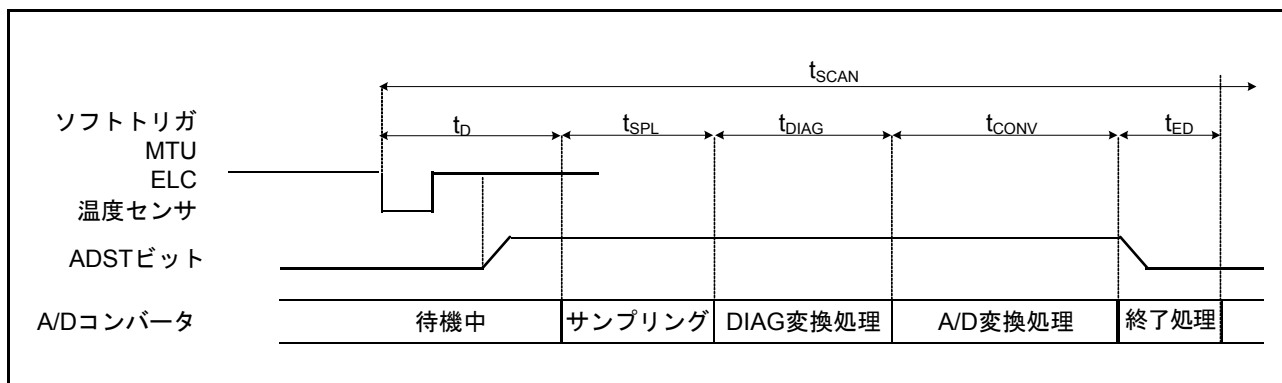
図 35.9 スキャン変換のタイミング (ソフトウェア起動、MTU、ELC、温度センサ起動の場合)
