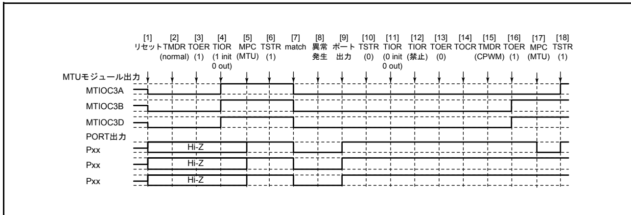
図 22.129 ノーマルモードで異常が発生し、相補 PWM モードで復帰する場合
