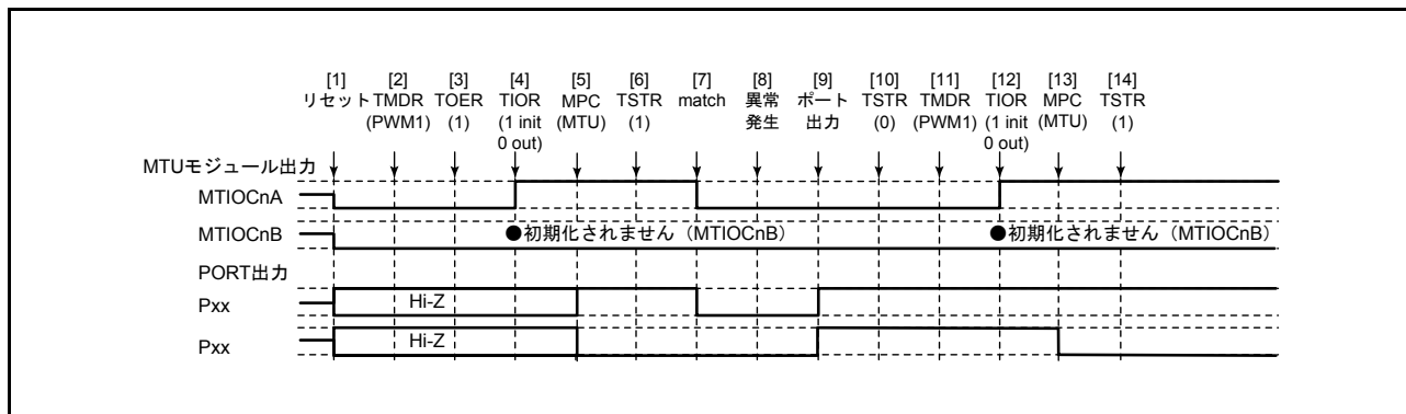
図 22.132 PWM モード 1 で異常が発生し、PWM モード 1 で復帰する場合
