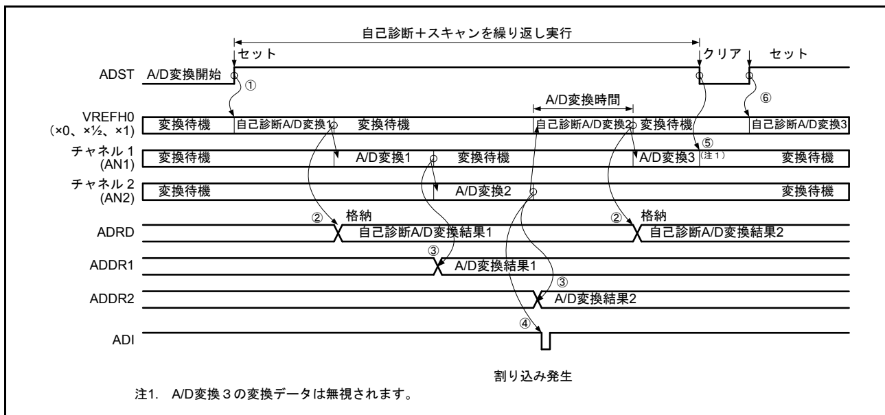
図 35.8 連続スキャンモードの動作 (基本動作+自己診断)
