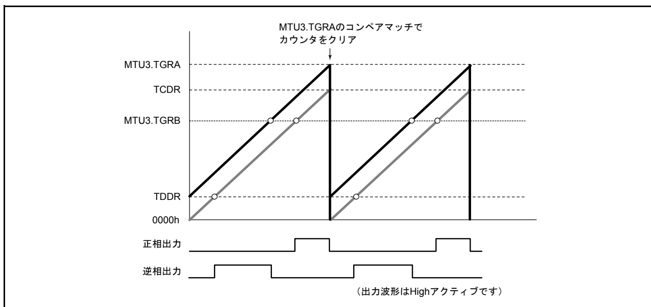
図 22.62 MTU3.TGRA のコンペアマッチにおけるカウンタクリアの動作例
