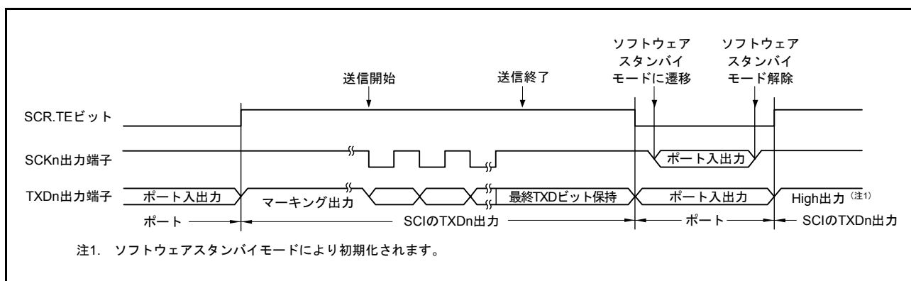
図 29.55 ソフトウェアスタンバイモード遷移時のポートの端子状態 (内部クロック、クロック同期送信)
