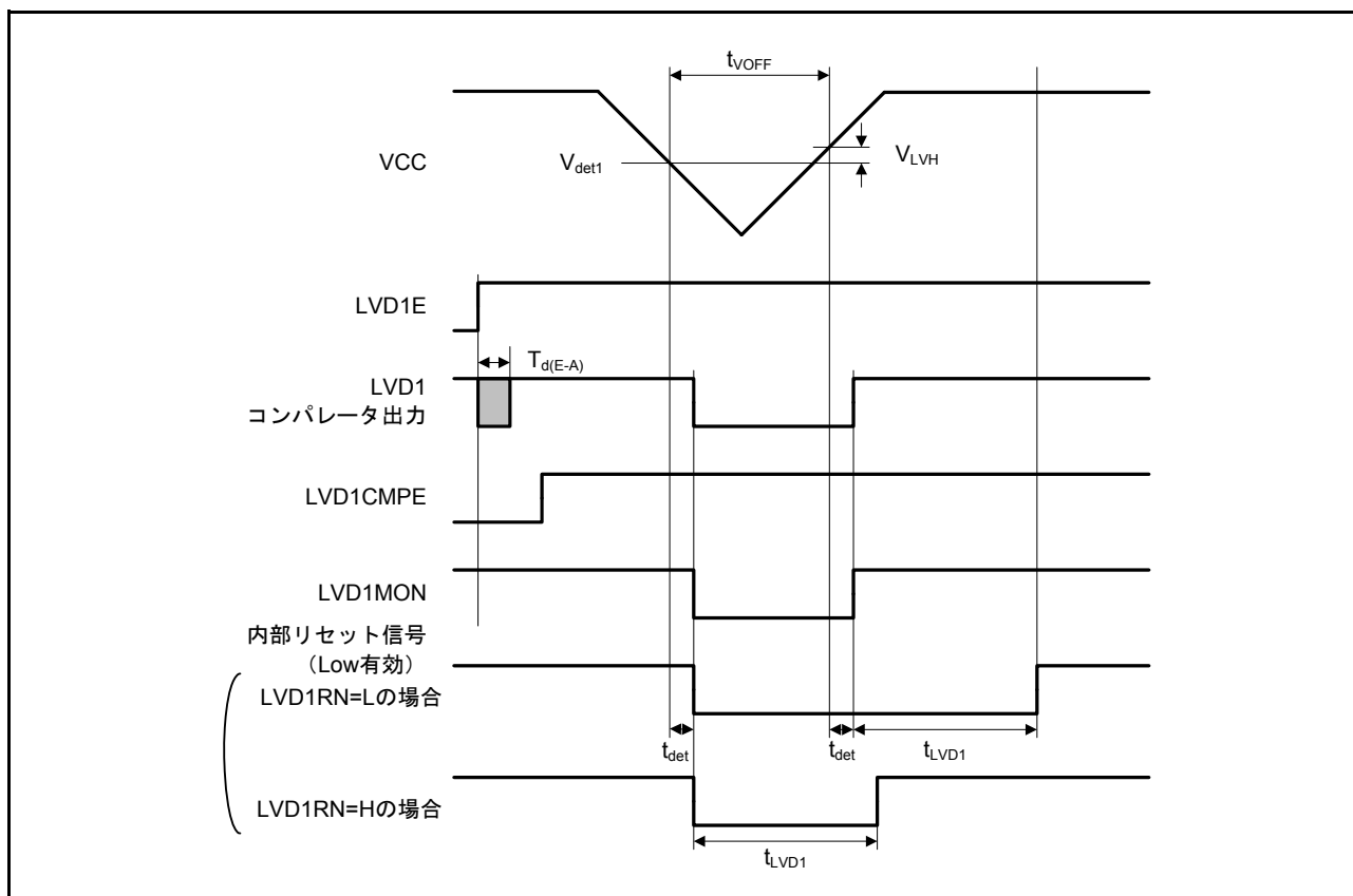
図 44.67 電圧検出回路タイミング (V det1 )
