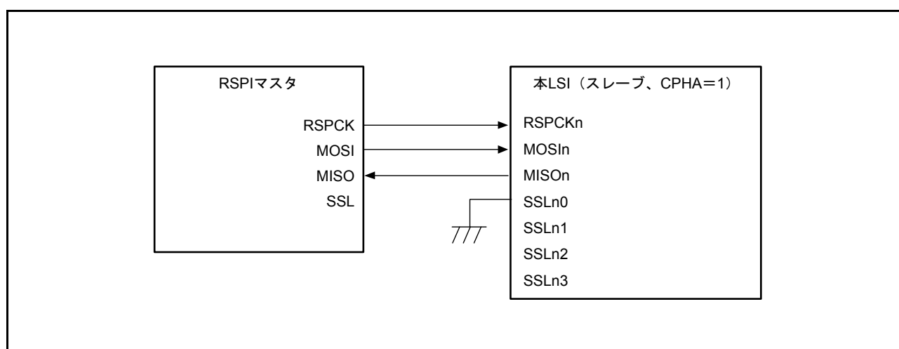
図 32.7 シングルマスタ / シングルスレーブの構成例 (本 LSI = スレーブ、CPHA = 1)
