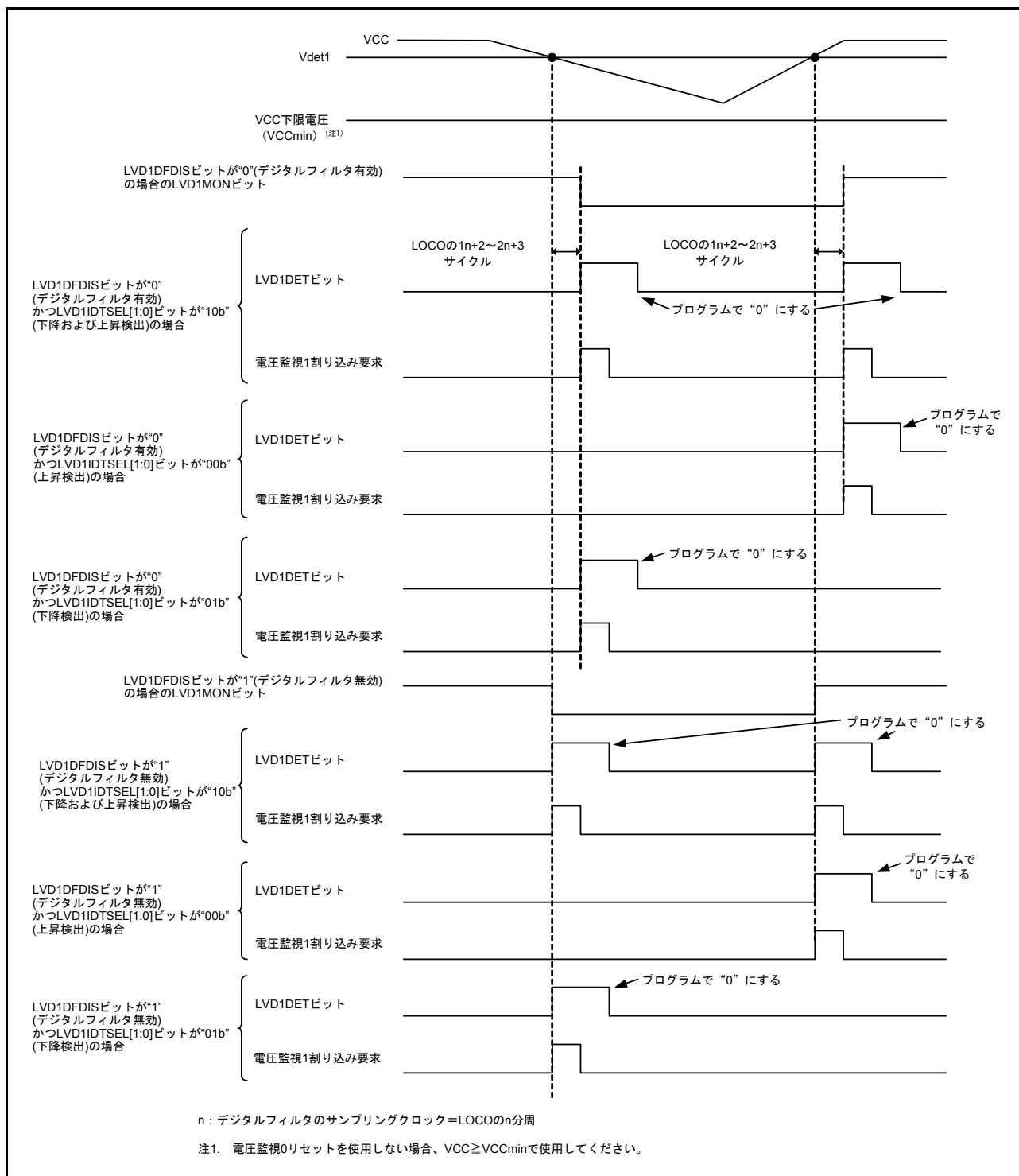
図 8.5 電圧監視 1 割り込み動作例
