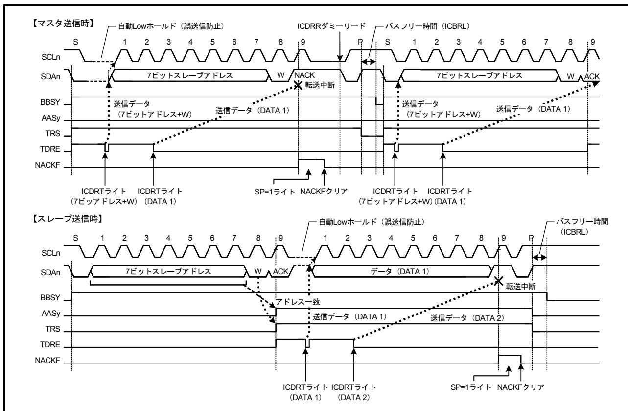
図 31.31 NACK 受信時の転送中断動作 (NACKC=1 のとき)
