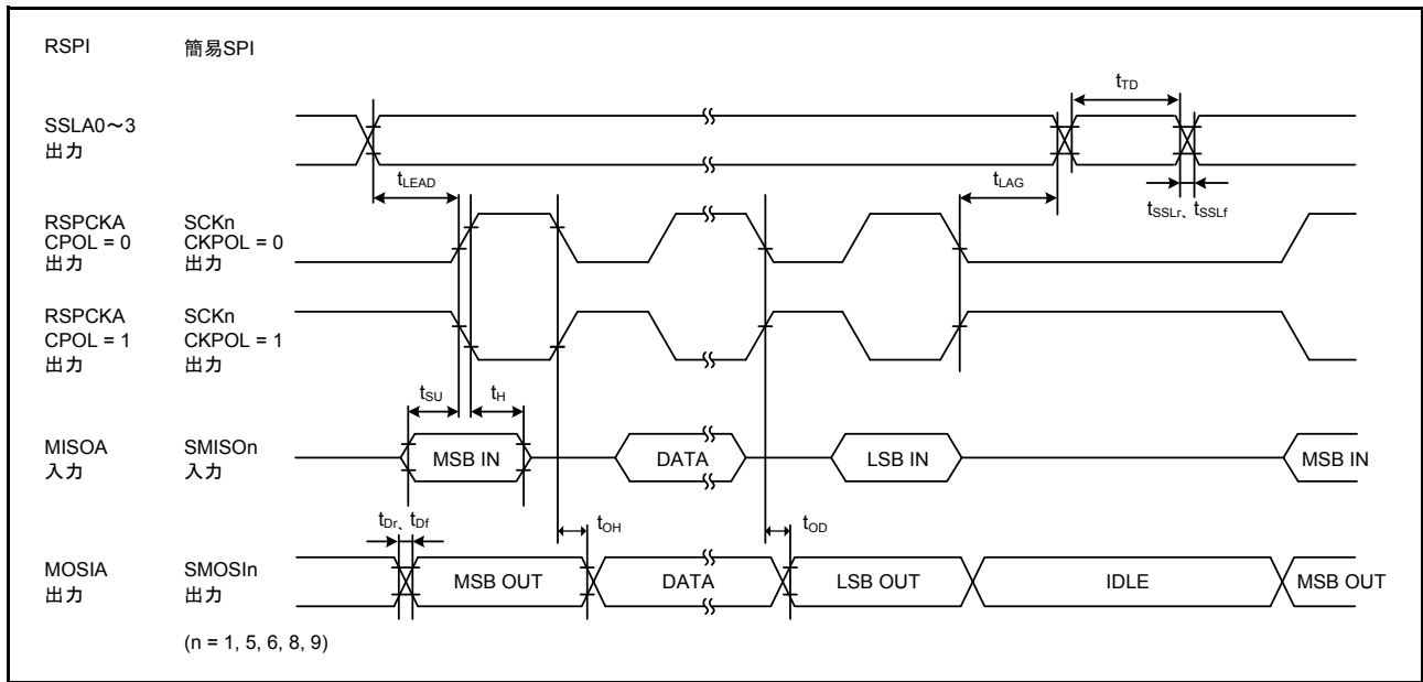
図 44.50 RSPI タイミング (マスタ、CPHA = 0) / 簡易 SPI タイミング (マスタ、CKPH = 1)
