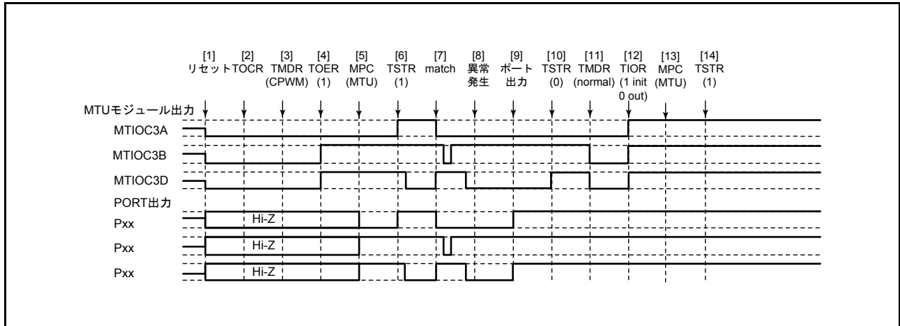
図 22.145 相補 PWM モードで異常が発生し、ノーマルモードで復帰する場合
