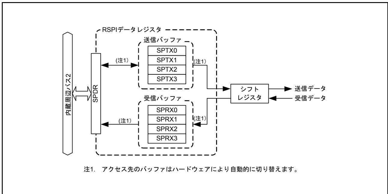
図 32.2 SPDR レジスタの構造図
