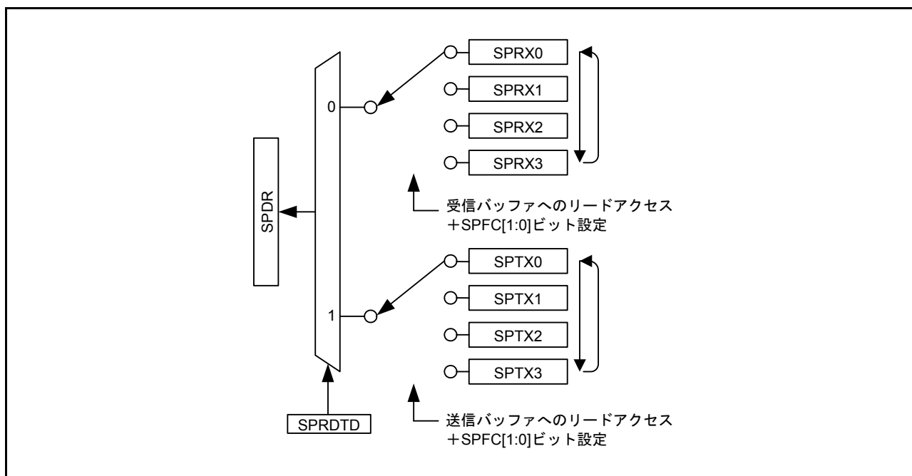
図 32.4 SPDR レジスタの構成図 (リード時)
