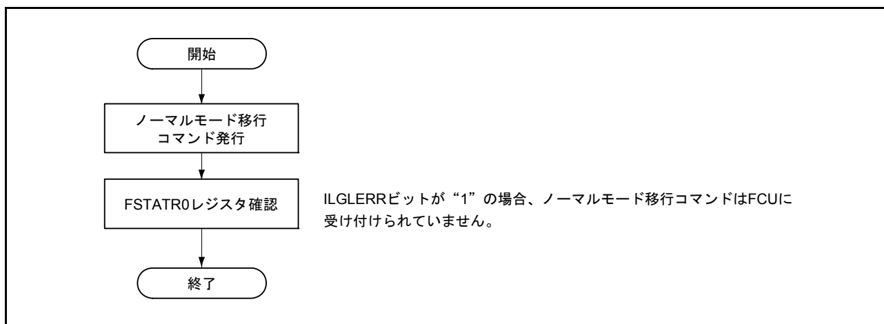
図 42.7 ROM P/E ノーマルモード移行フロー
