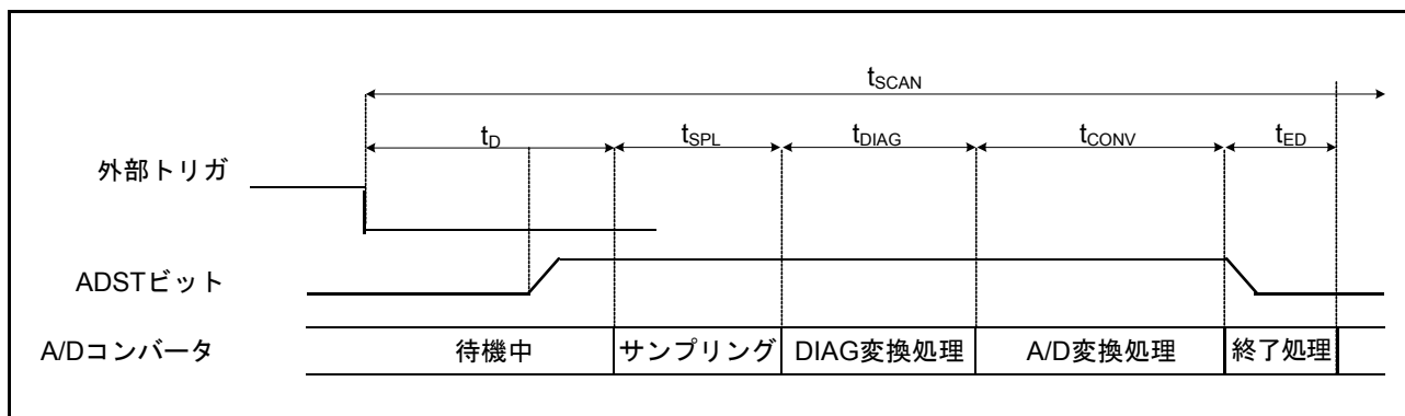
図 35.10 スキャン変換のタイミング (ADTRG0# 要因の場合)
