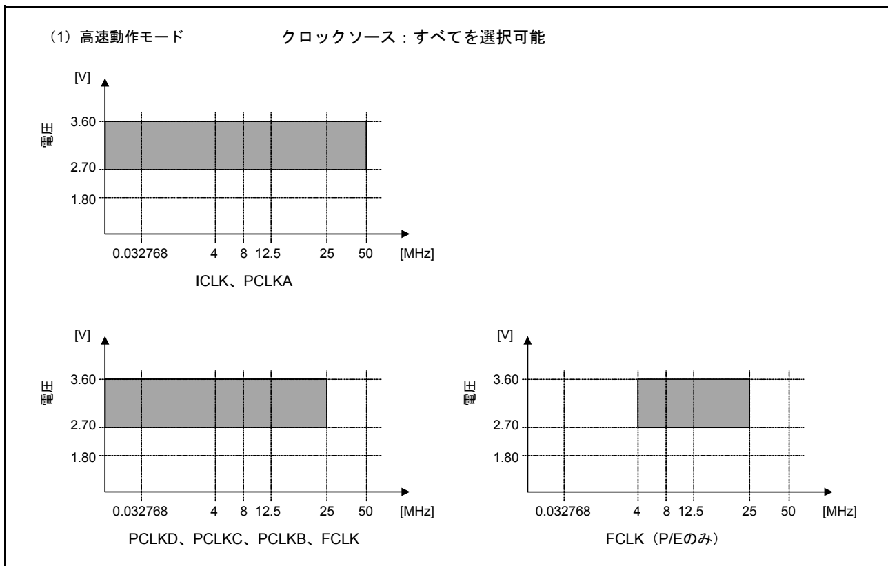
図 11.2 高速動作モードにおける動作電圧と動作周波数の関係
