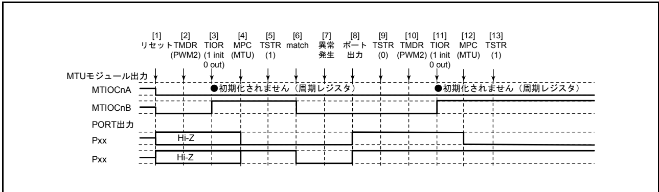
図 22.139 PWM モード 2 で異常が発生し、PWM モード 2 で復帰する場合
