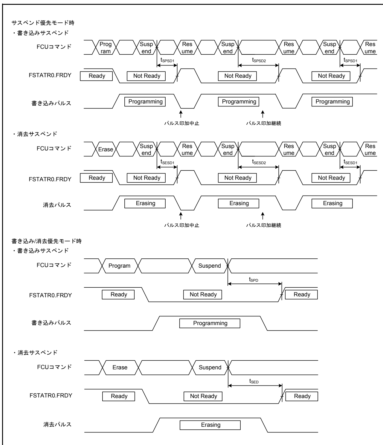
図 44.70 フラッシュメモリプログラム/イレーズサスペンドタイミング
