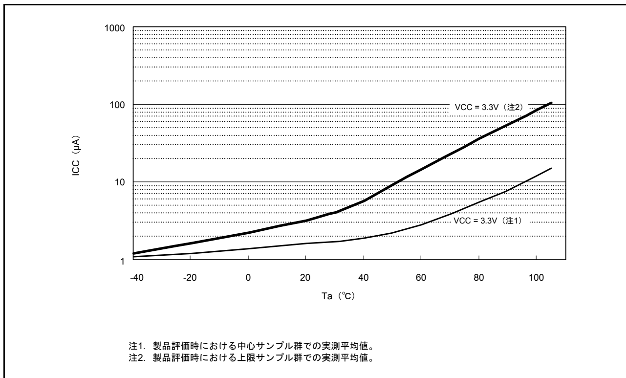
図 44.7 ソフトウェアスタンバイモード (SOFTCUT[2:0] ビット = 110b) 時の温度依存性 (参考データ)
