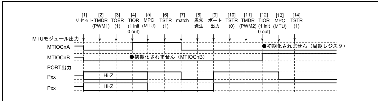
図 22.133 PWM モード 1 で異常が発生し、PWM モード 2 で復帰する場合
