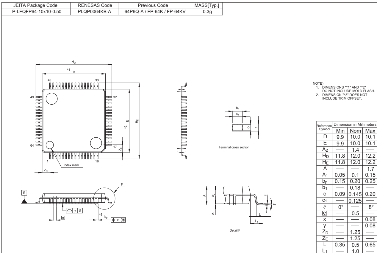
図 C. 64ピンLQFP (PLQP0064KB-A)
