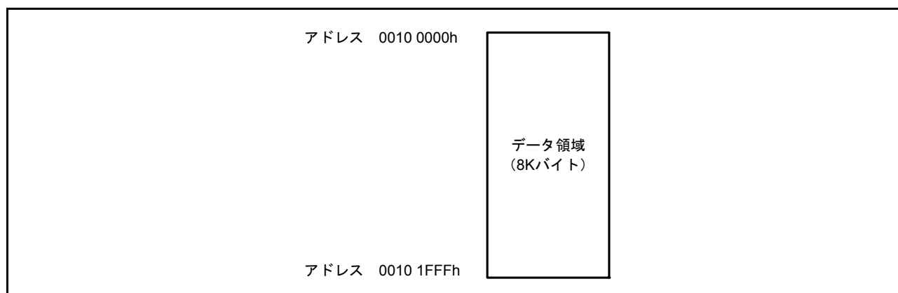
図 43.2 E2データフラッシュのデータ領域構成
