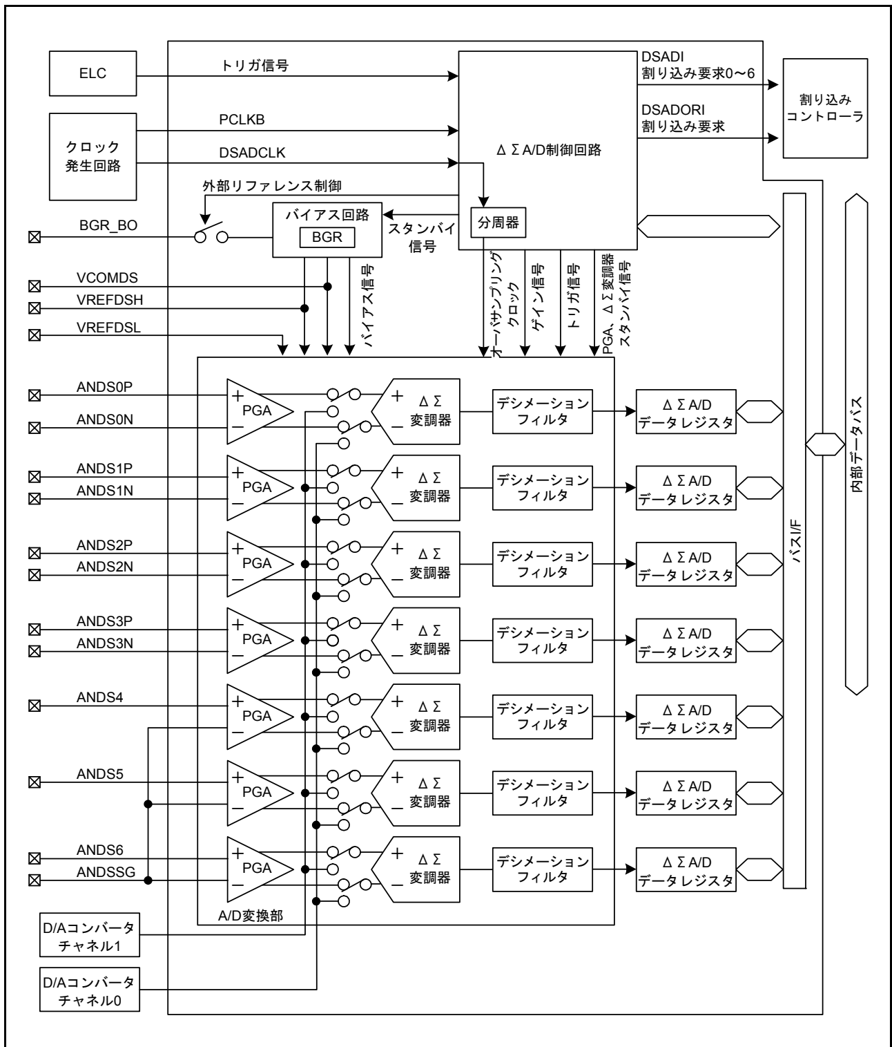
図 34.1 \Delta\Sigma A/Dコンバータのブロック図
