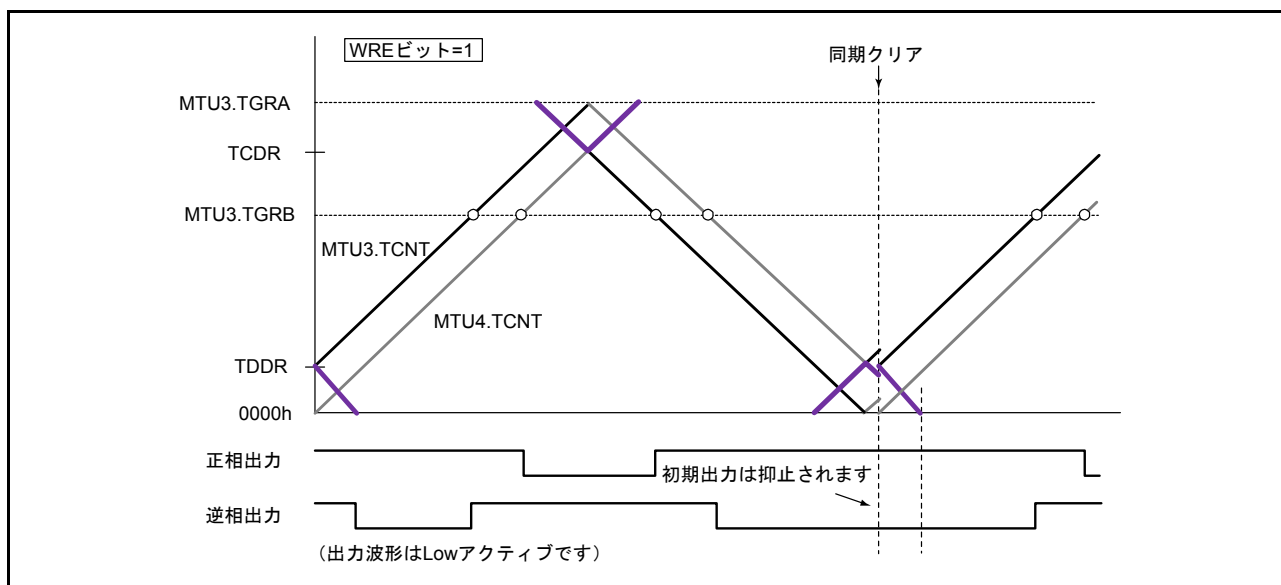
図 22.61 谷の Tb 区間で同期クリアが発生した場合 (図 22.56 のタイミング①、TWCR レジスタの WRE ビット=“1”)
