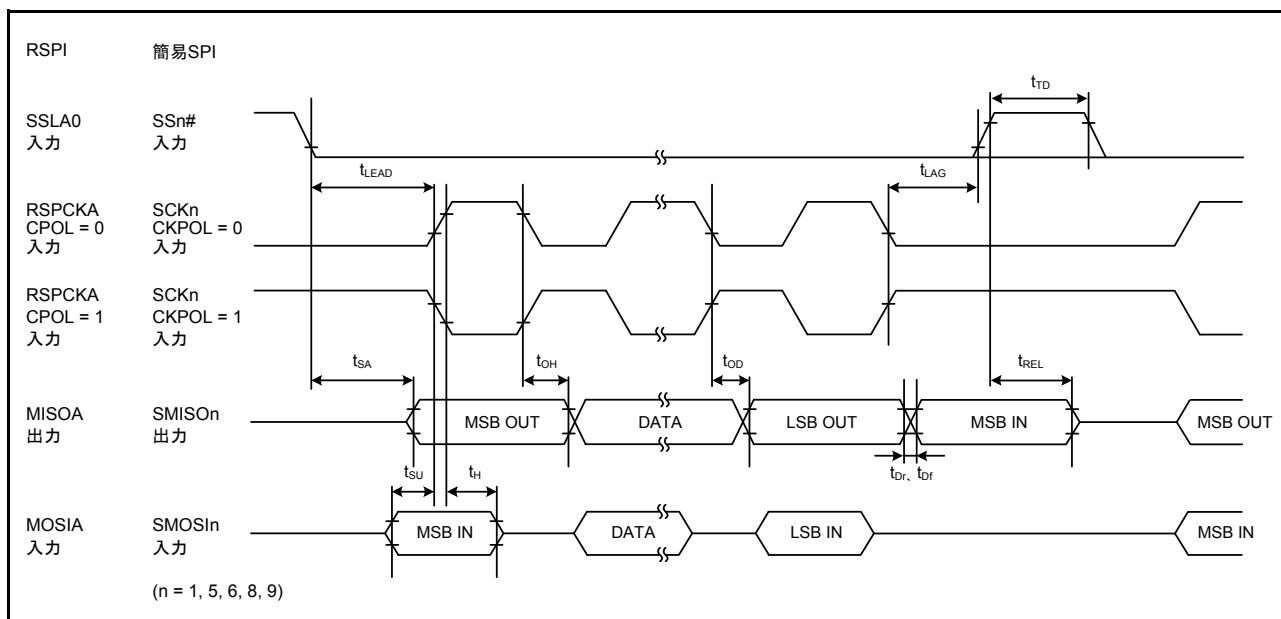
図 44.52 RSPI タイミング (スレーブ、CPHA = 0) / 簡易 SPI タイミング (スレーブ、CKPH = 1)
