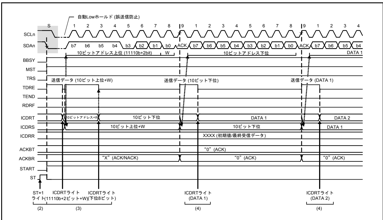
図 31.8 マスタ送信の動作タイミング (2) (10ビットアドレスフォーマットのとき)
