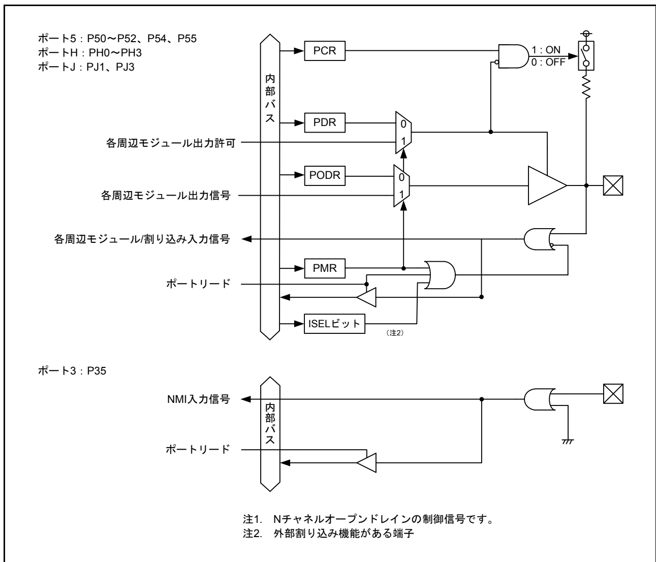
図 20.3 入出力ポートの構成 (3)
