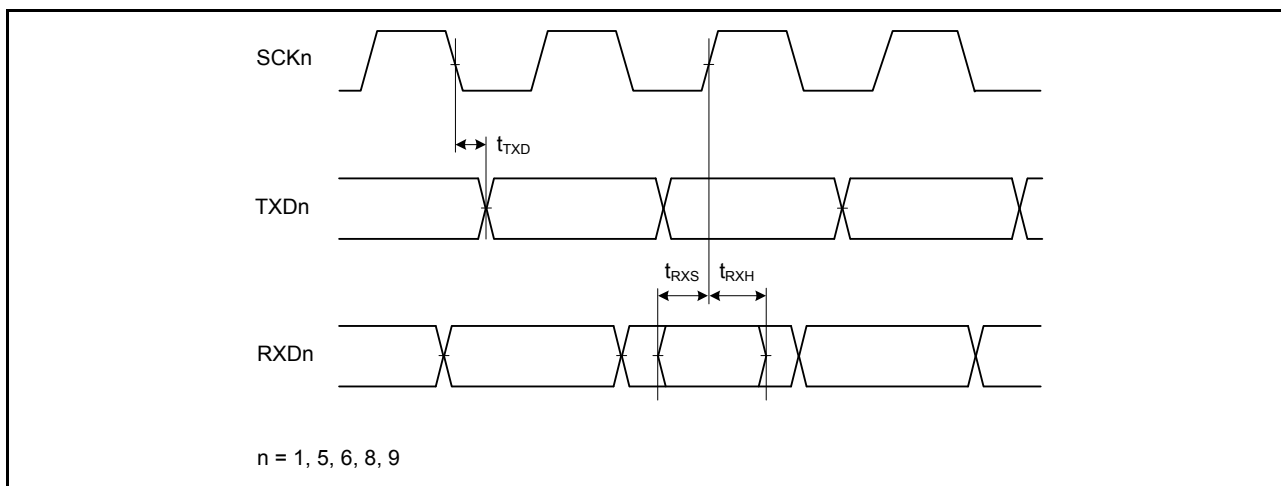
図 44.47 SCI 入出力タイミング / クロック同期式モード
