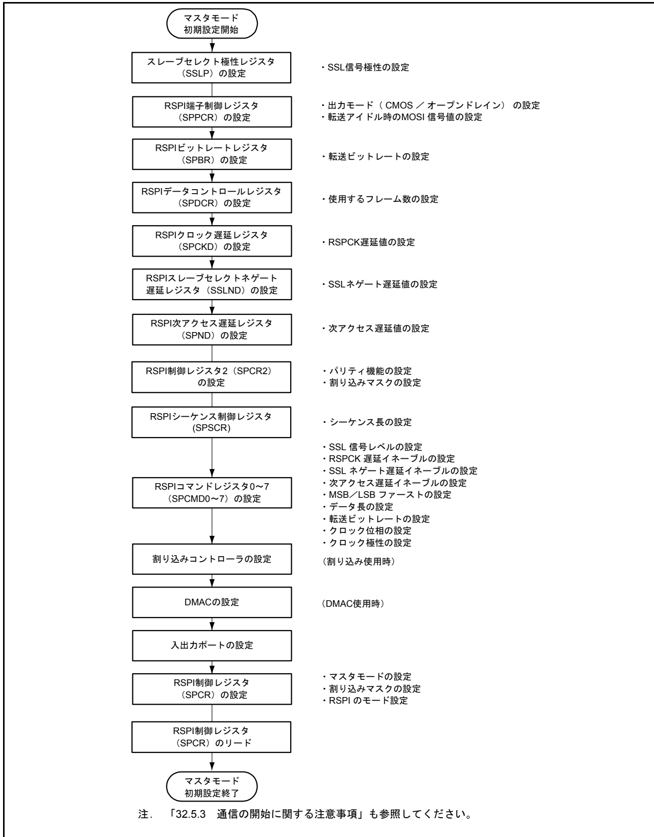
図 32.34 マスタモード時の初期化フロー例 (SPI 動作)
