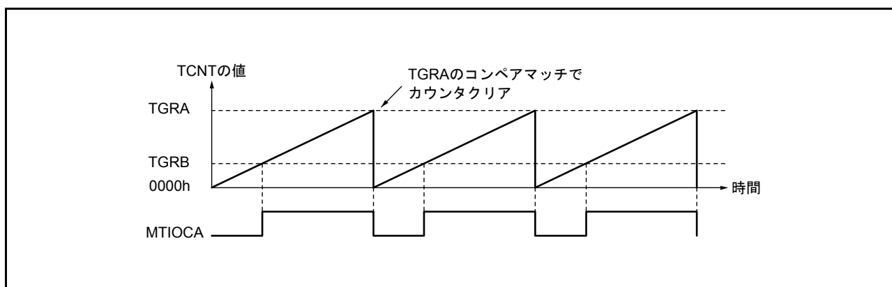
図 22.26 PWM モードの動作例
