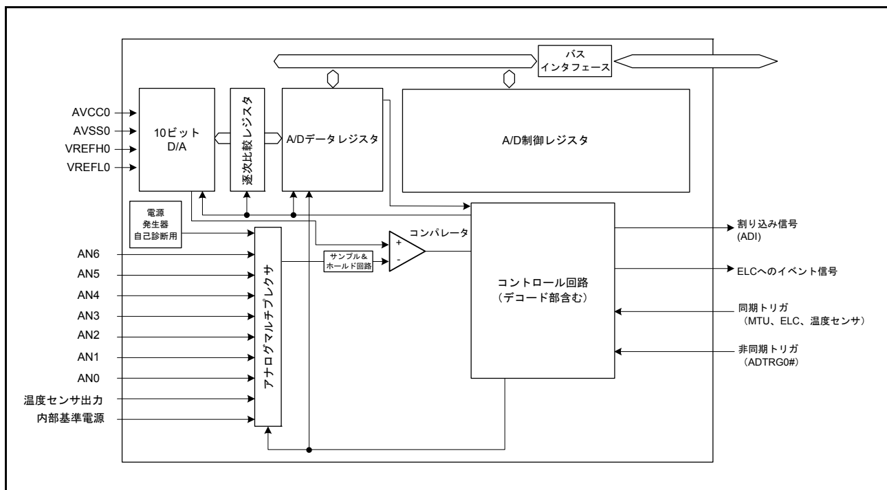
図 35.1 10ビットA/Dコンバータのブロック図
