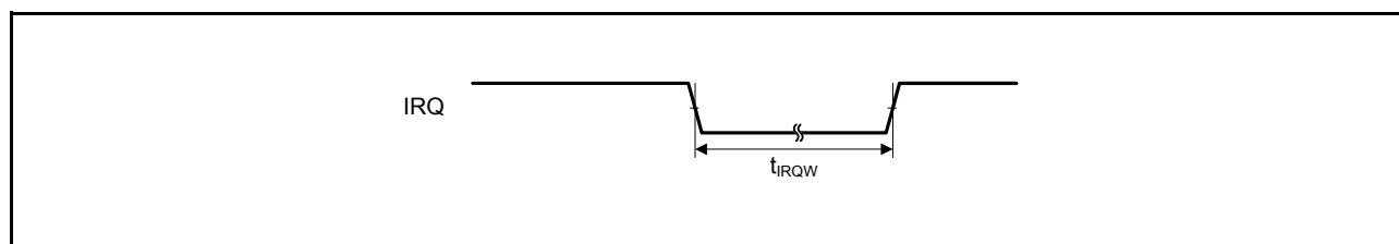
図 44.40 IRQ 割り込み入カタイミング
