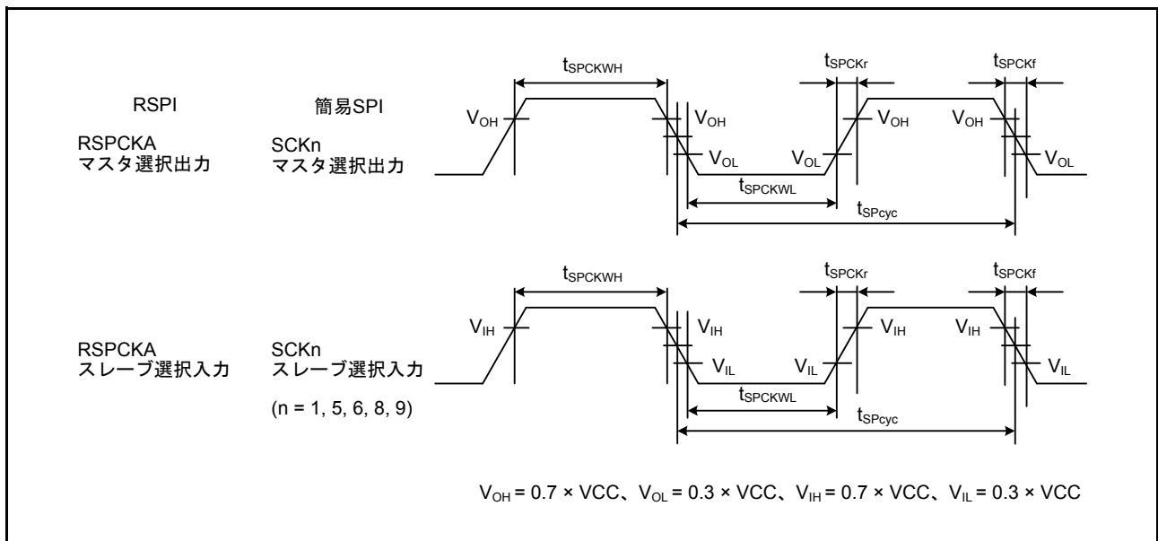
図 44.49 RSPI クロックタイミング / 簡易 SPI クロックタイミング
