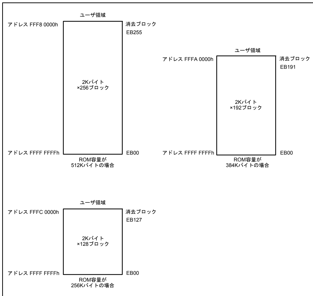
図 42.3 ユーザ領域の消去ブロックの構成
