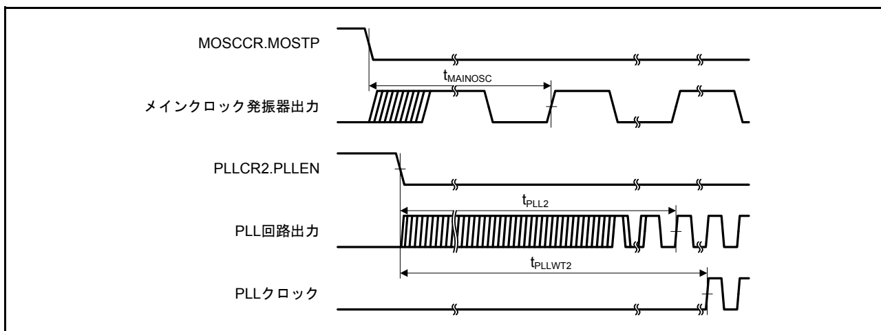
図 44.32 PLL クロック発振開始タイミング (メインクロック発振安定を待たずに PLL を動作させたとき)
