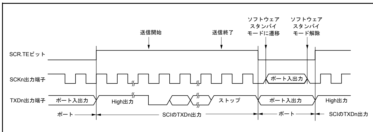
図 29.54 ソフトウェアスタンバイモード遷移時のポートの端子状態 (内部クロック、調歩同期送信)
