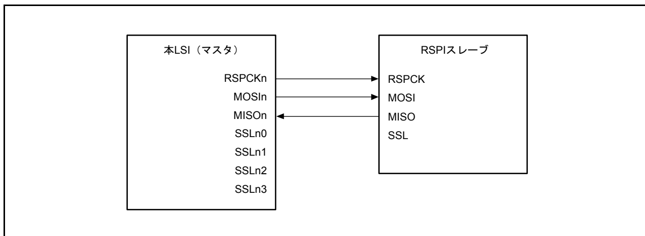
図 32.11 マスタ (クロック同期式動作) / スレーブ (クロック同期式動作) の構成例 (本 LSI = マスタ)
