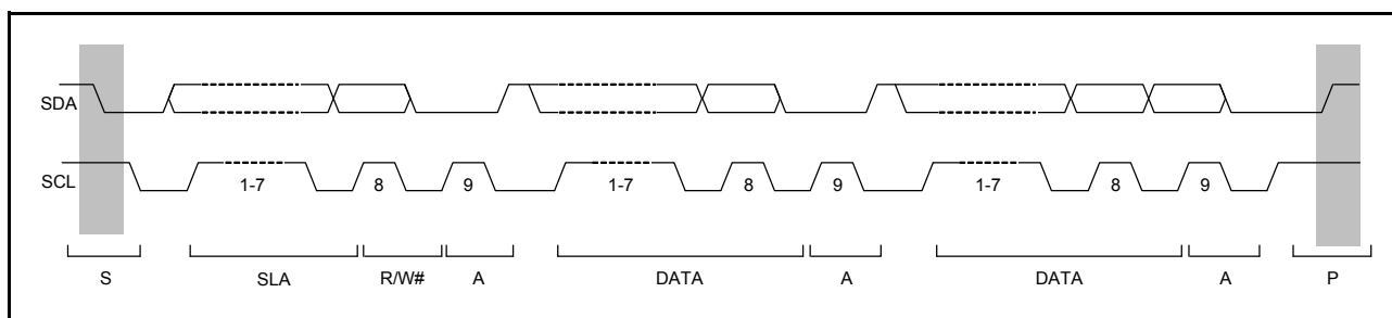
図 31.4 I 2 C バスタイミング (SLA=7 ビットの場合)
