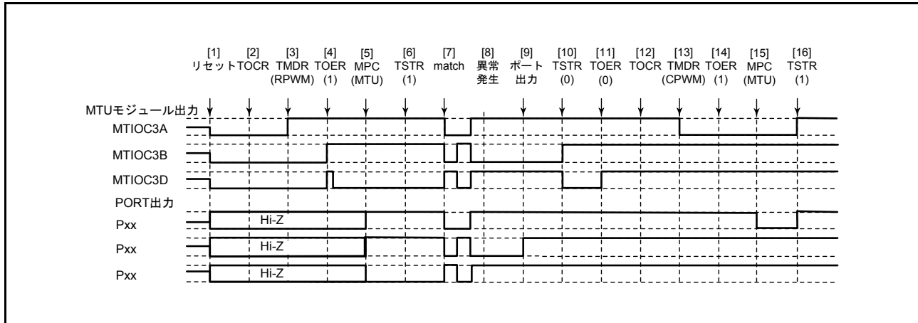
図 22.152 リセット同期 PWM モードで異常が発生し、相補 PWM モードで復帰する場合
