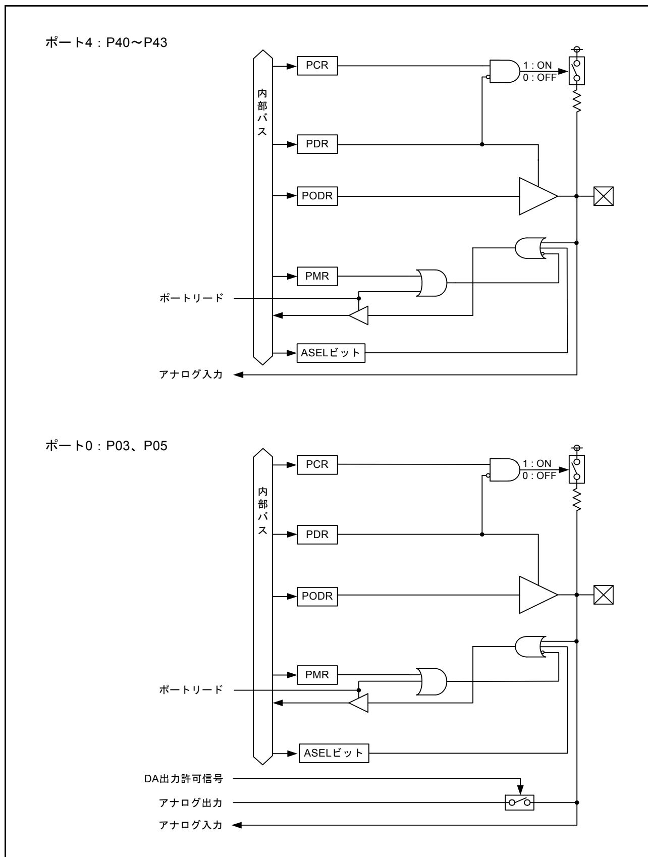
図 20.1 入出力ポートの構成 (1)
