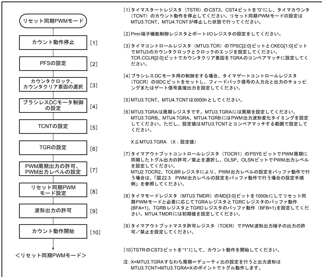
図 22.35 リセット同期 PWM モードの設定手順例
