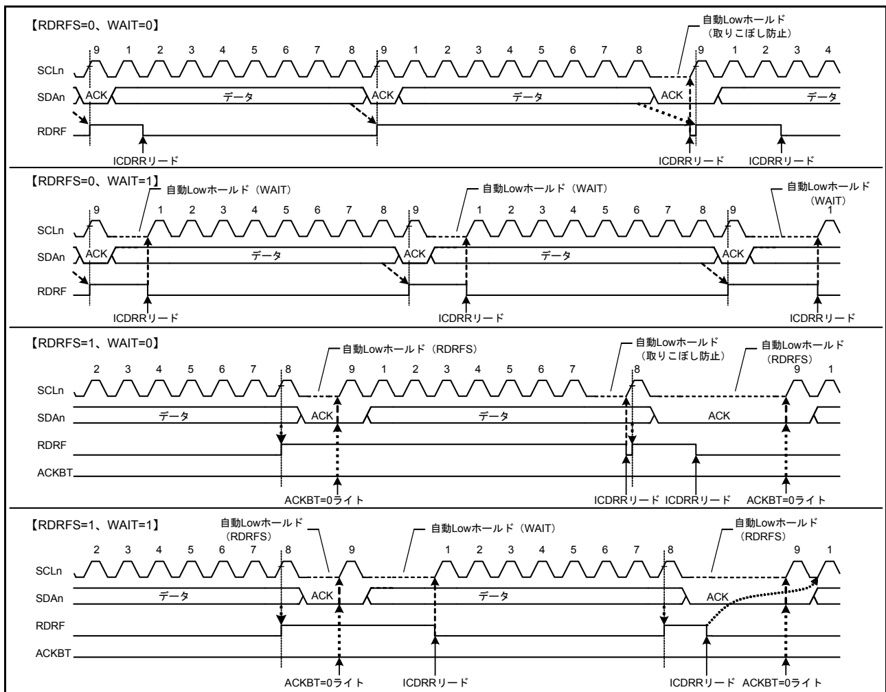
図 31.32 受信モードの自動 Low ホールド動作 (RDRFS、WAIT ビット)
