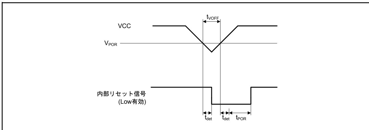
図 44.64 電圧検出リセットタイミング
