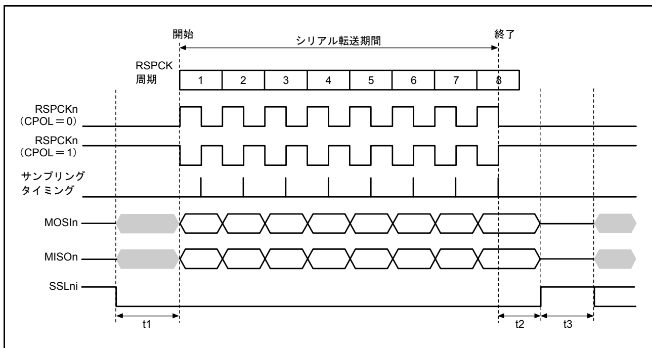
図 32.24 RSPI 転送フォーマット (CPHA ビット = 1)
