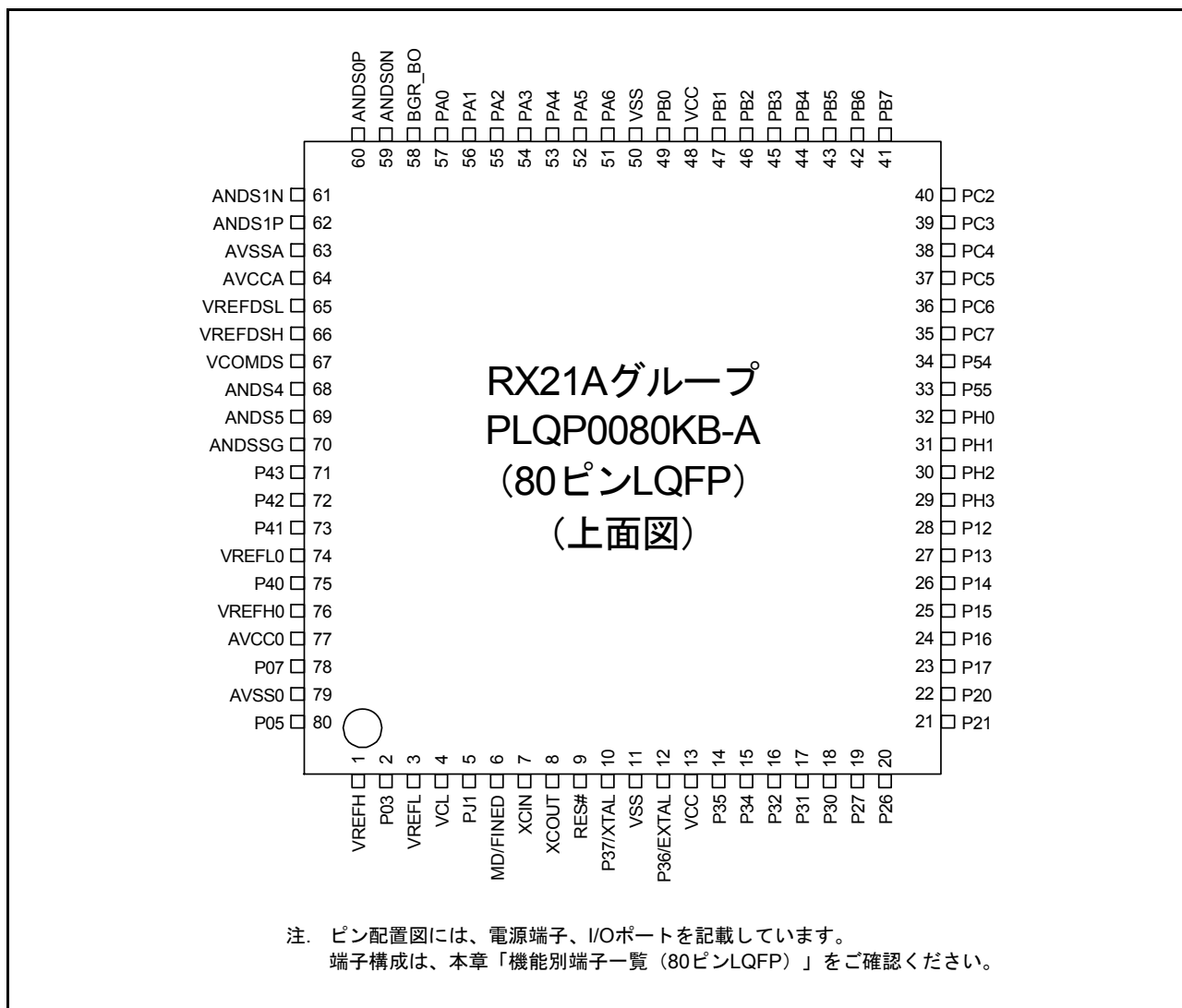
図 1.4 80 ピン LQFP ピン配置図
