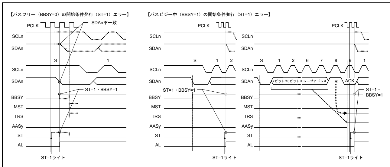
図 31.34 スタートコンディション発行時のアービトレーションロスト (MALE=1 のとき)
