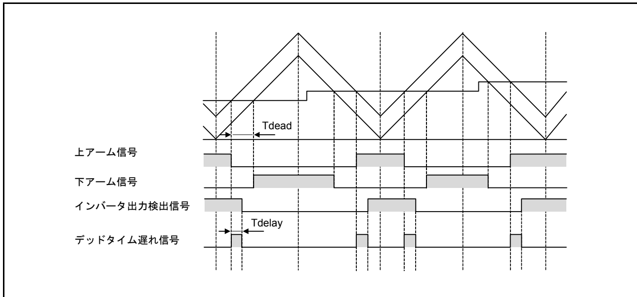
図 22.79 相補 PWM モード動作時のデッドタイム遅れ
