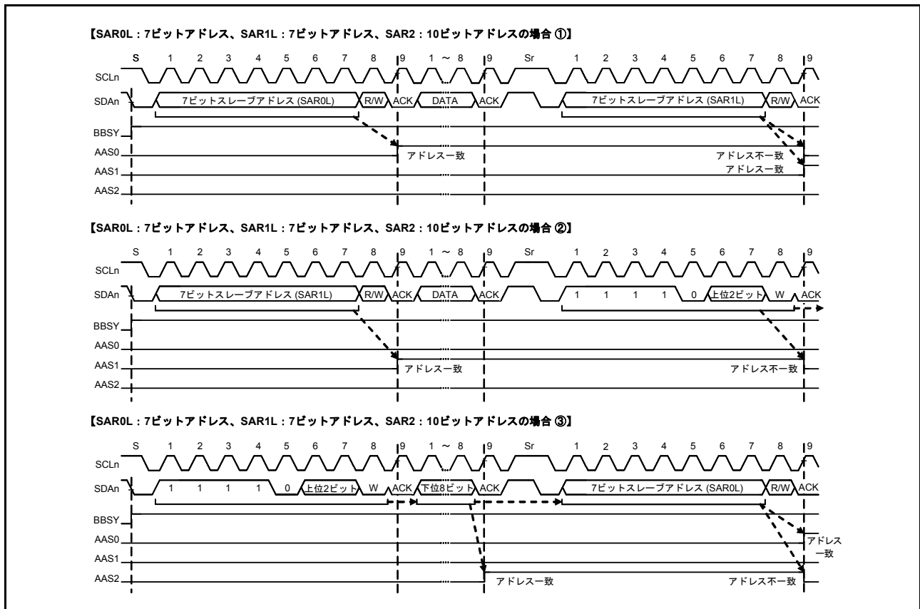
図 31.26 7ビット/10ビットアドレスフォーマット混在時に AASy フラグが“1”/“0”になるタイミング
