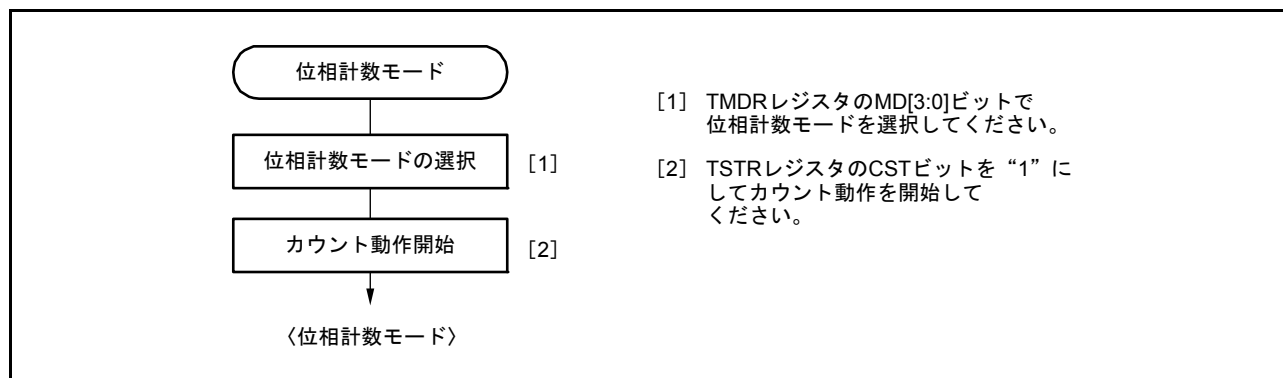
図 22.29 位相計数モードの設定手順例
