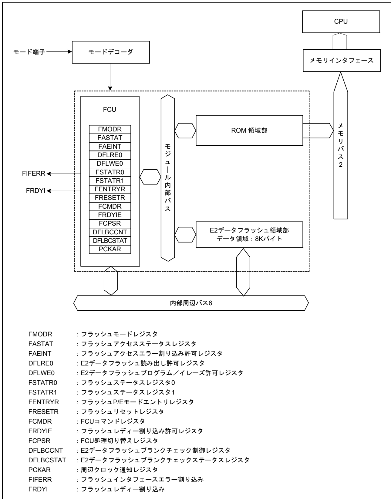
図 43.1 E2 データフラッシュのブロック図
