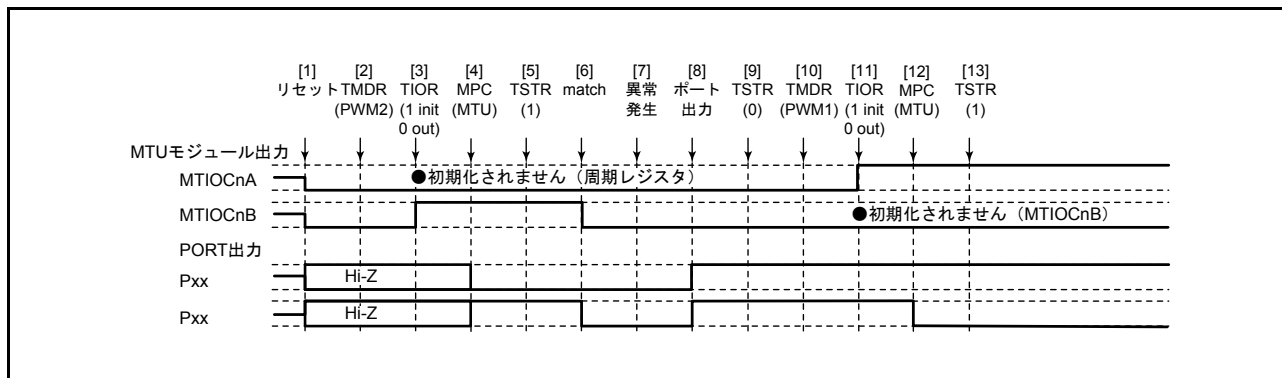
図 22.138 PWM モード 2 で異常が発生し、PWM モード 1 で復帰する場合
