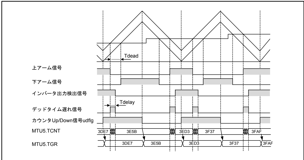
図 22.82 相補 PWM モード時の「山/谷」での MTU5.TCNT キャプチャ動作
