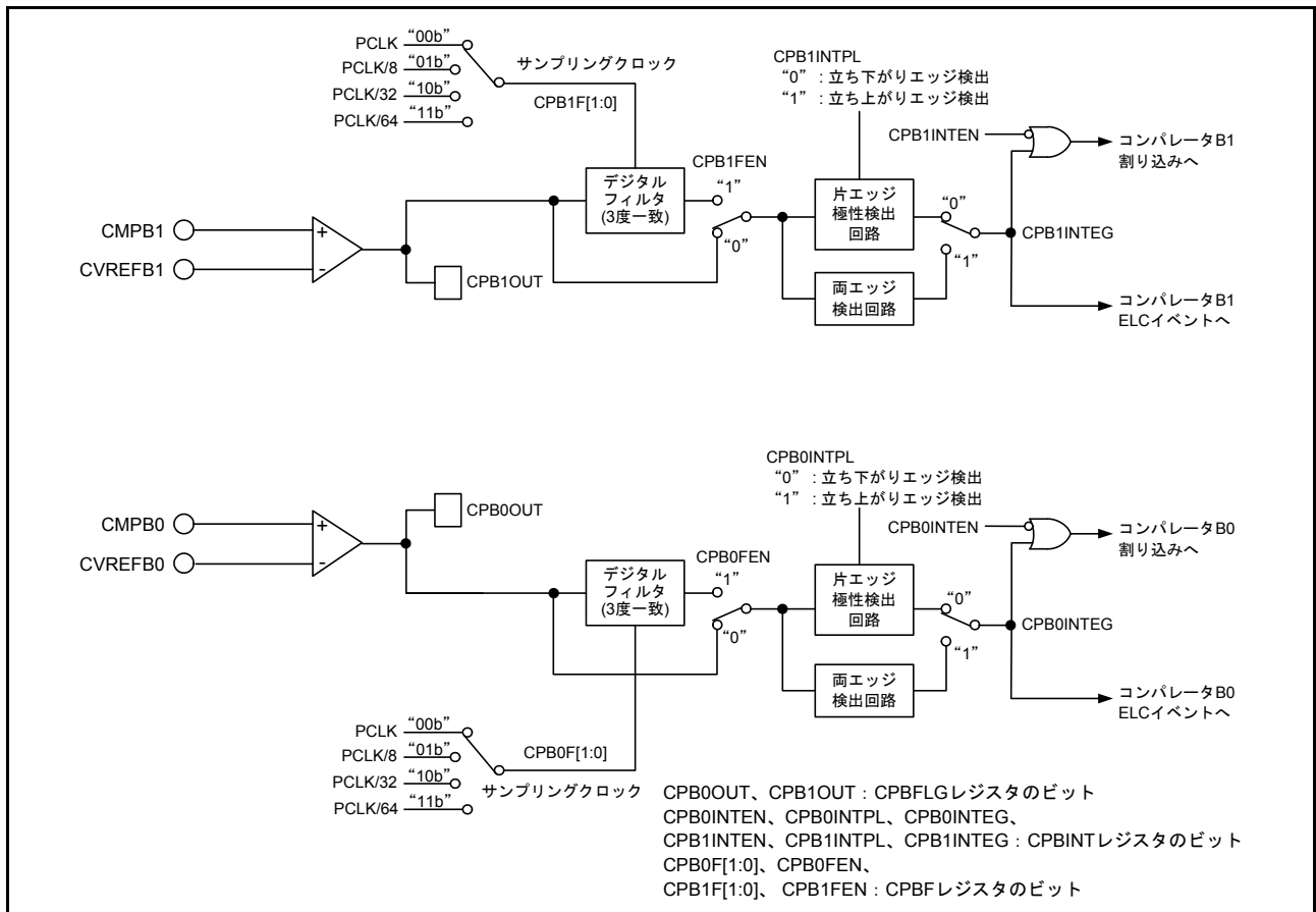
図 39.1 コンパレータ B のブロック図
