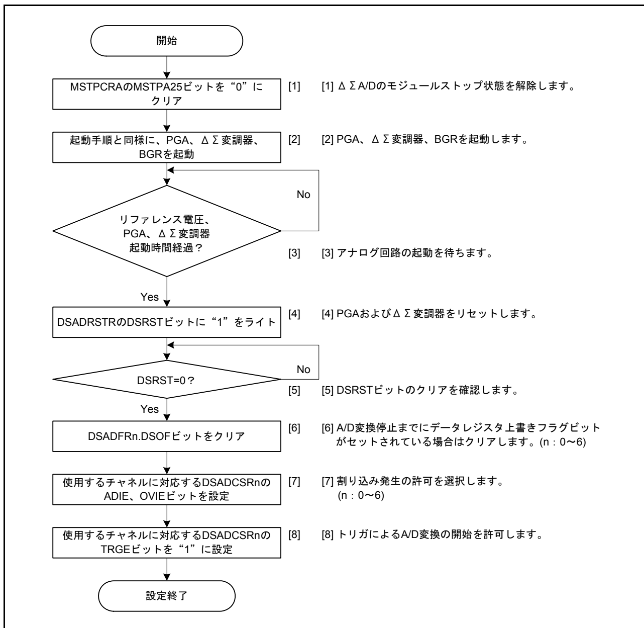
図 34.4 \Delta\Sigma A/Dコンバータの再開手順
