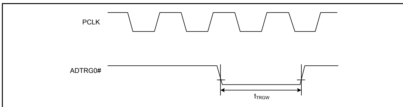
図 44.48 A/D コンバータ外部トリガ入力タイミング
