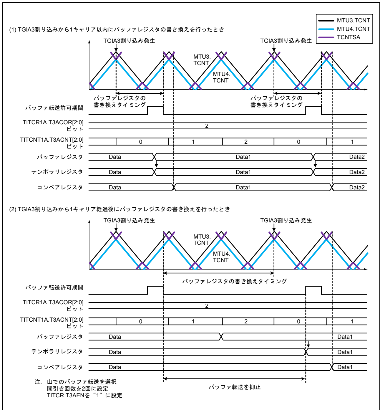
図 22.71 バッファ転送を割り込み間引きと連動する設定 (BTE[1:0] = “10b”) にした場合の動作例
