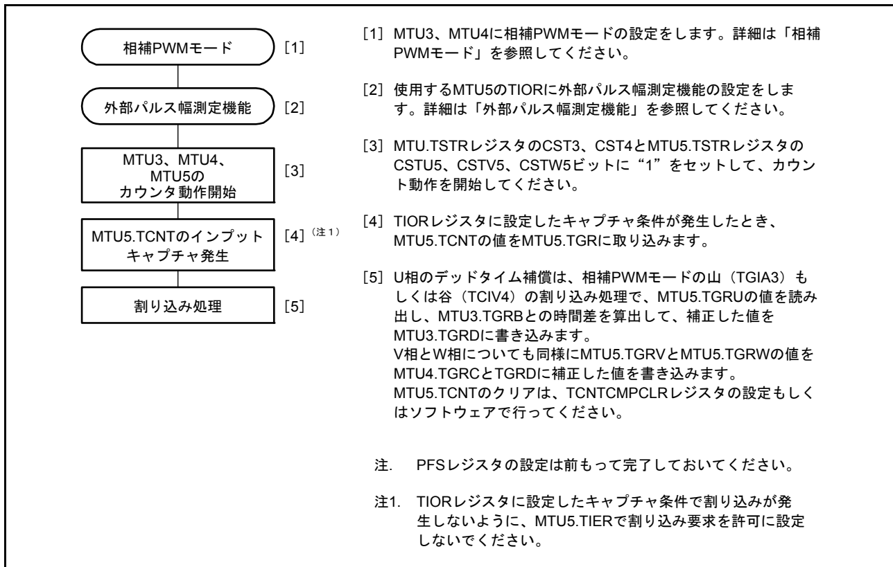
図 22.80 デッドタイム補償機能の設定手順例
