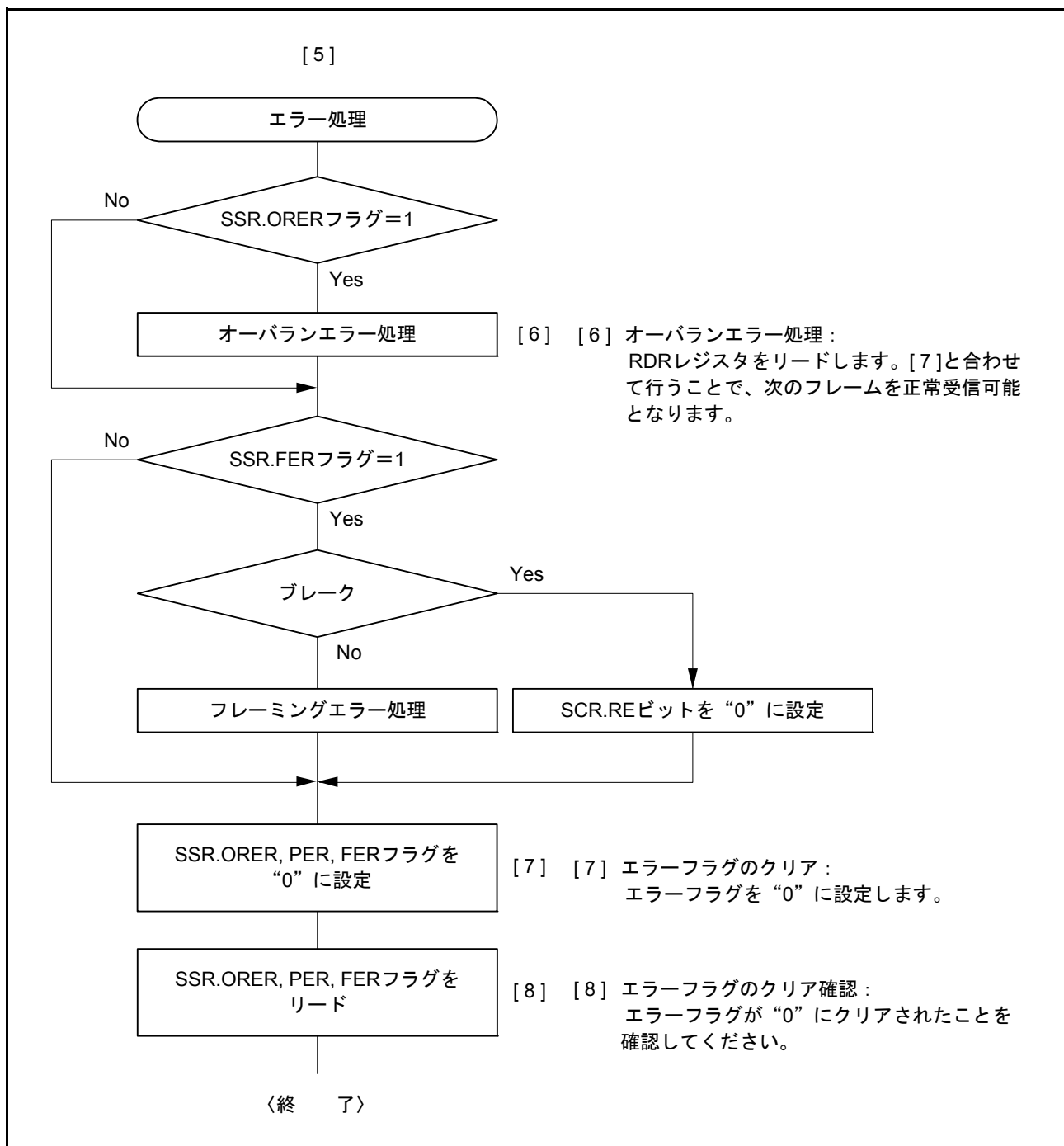
図 29.18 マルチプロセッサシリアル受信のフローチャートの例 (2)
