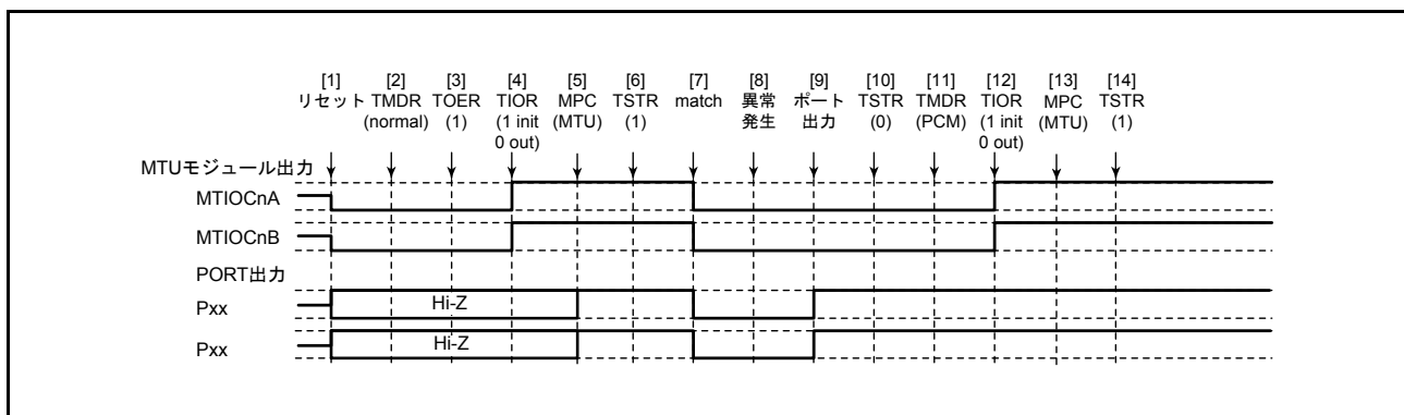
図 22.128 ノーマルモードで異常が発生し、位相計数モードで復帰する場合
