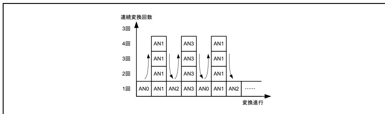
図 35.2 ADADC.ADC[1:0] = 11b、ADS[1] = 1、ADS[3] = 1 選択時のスキャン変換シーケンス
