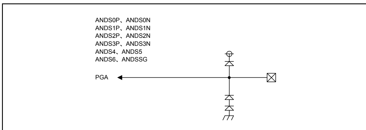
図 20.7 入出力ポートの構成 (7)
