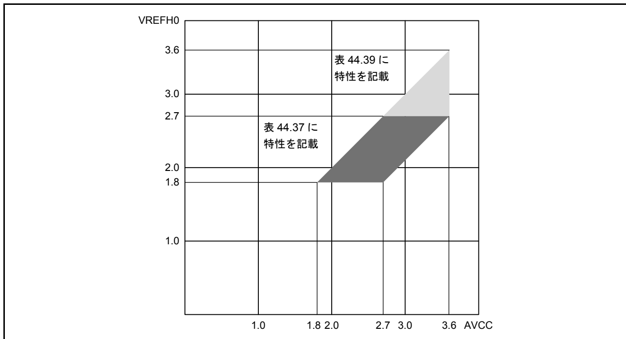
図 44.61 AVCC - VREFH0 電圧範囲
