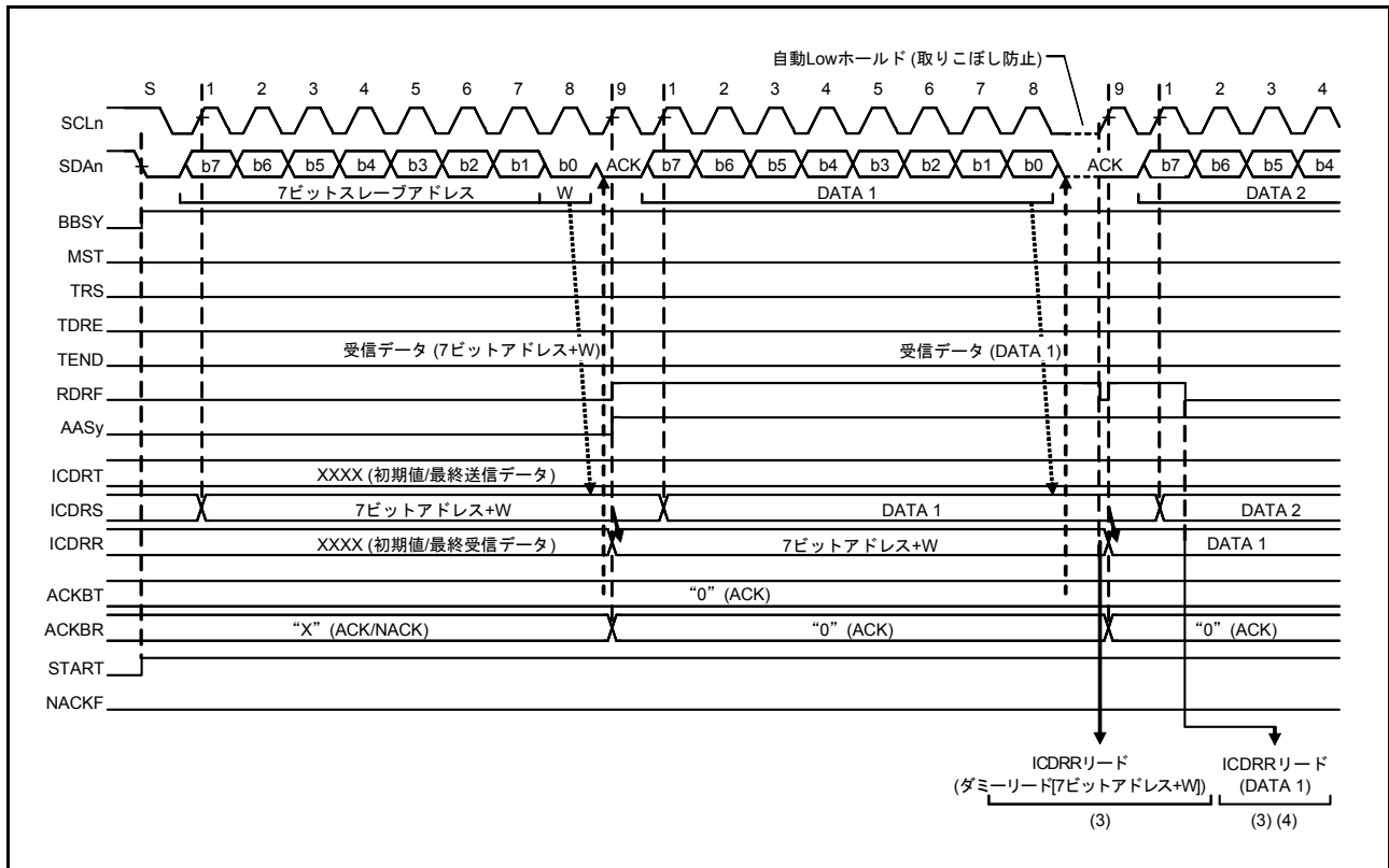
図 31.19 スレーブ受信の動作タイミング (1) (7ビットアドレスフォーマット、RDRFS=0 のとき)
