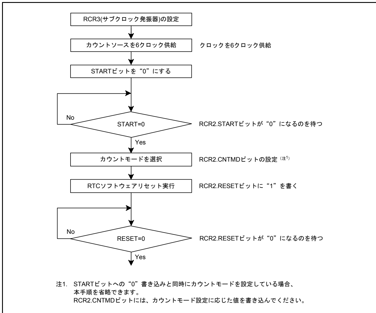
図 26.3 クロックとカウントモードの設定手順
