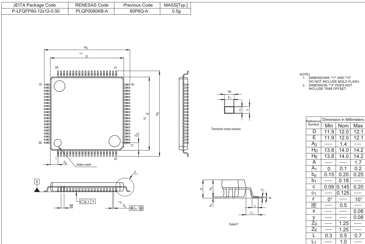
図 B. 80ピンLQFP (PLQP0080KB-A)
