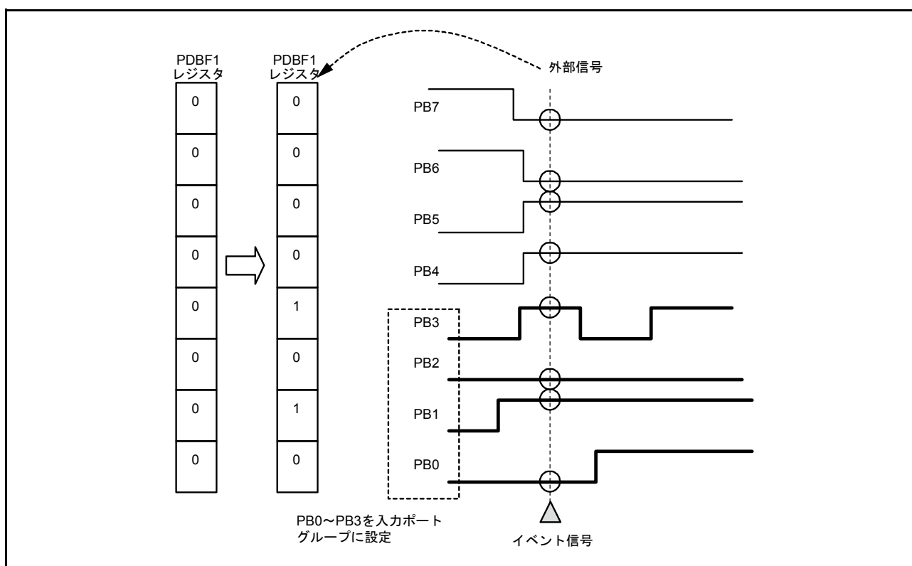
図 19.4 入力ポートグループのイベントリンク動作
