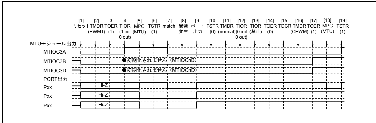
図 22.135 PWM モード 1 で異常が発生し、相補 PWM モードで復帰する場合
