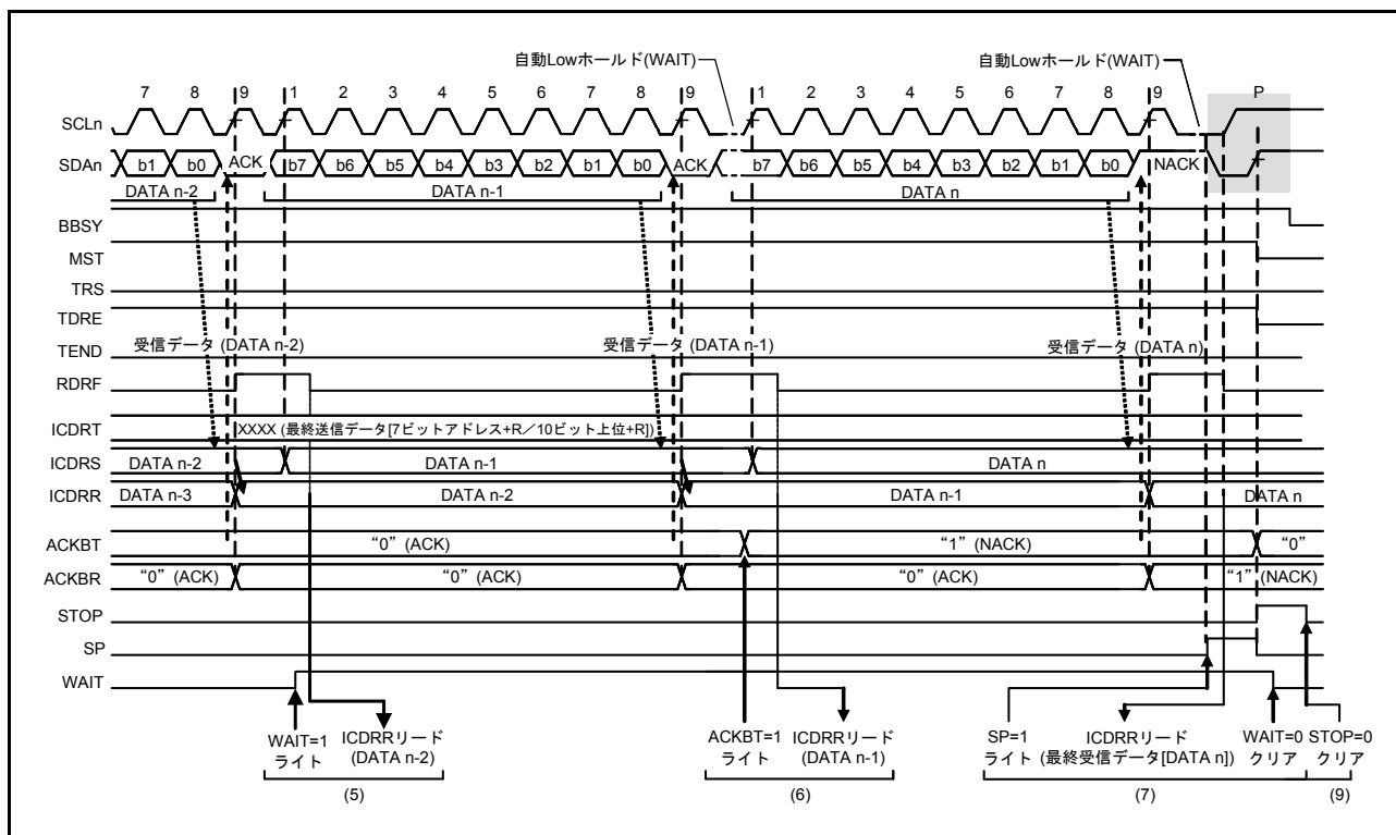
図 31.14 マスタ受信の動作タイミング (3) (RDRFS=0 のとき)
