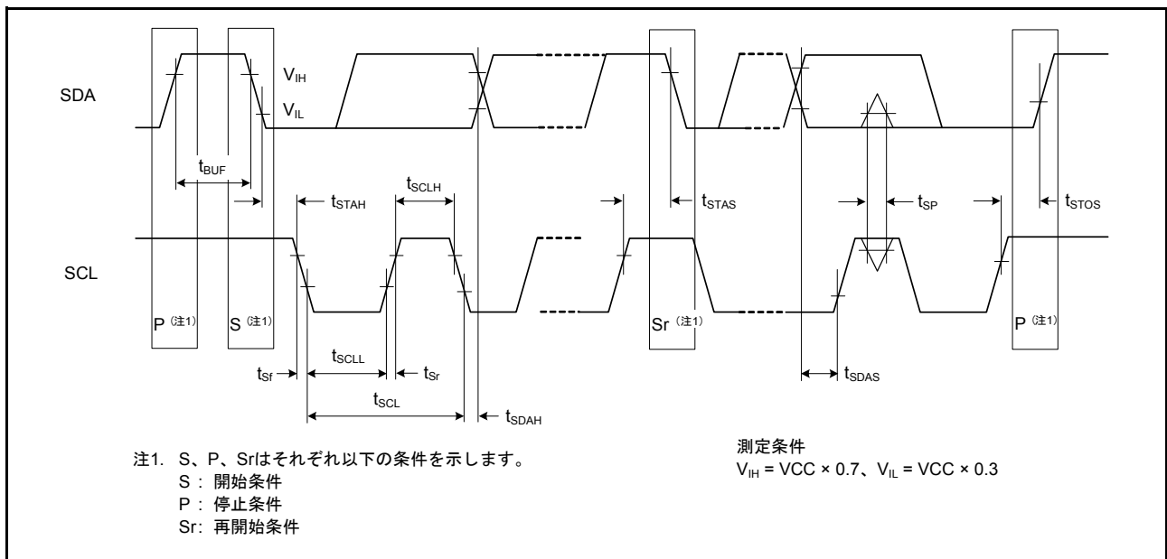
図 44.54 RIIC バスインタフェース入出力タイミング / 簡易 IIC バスインタフェース入出力タイミング
