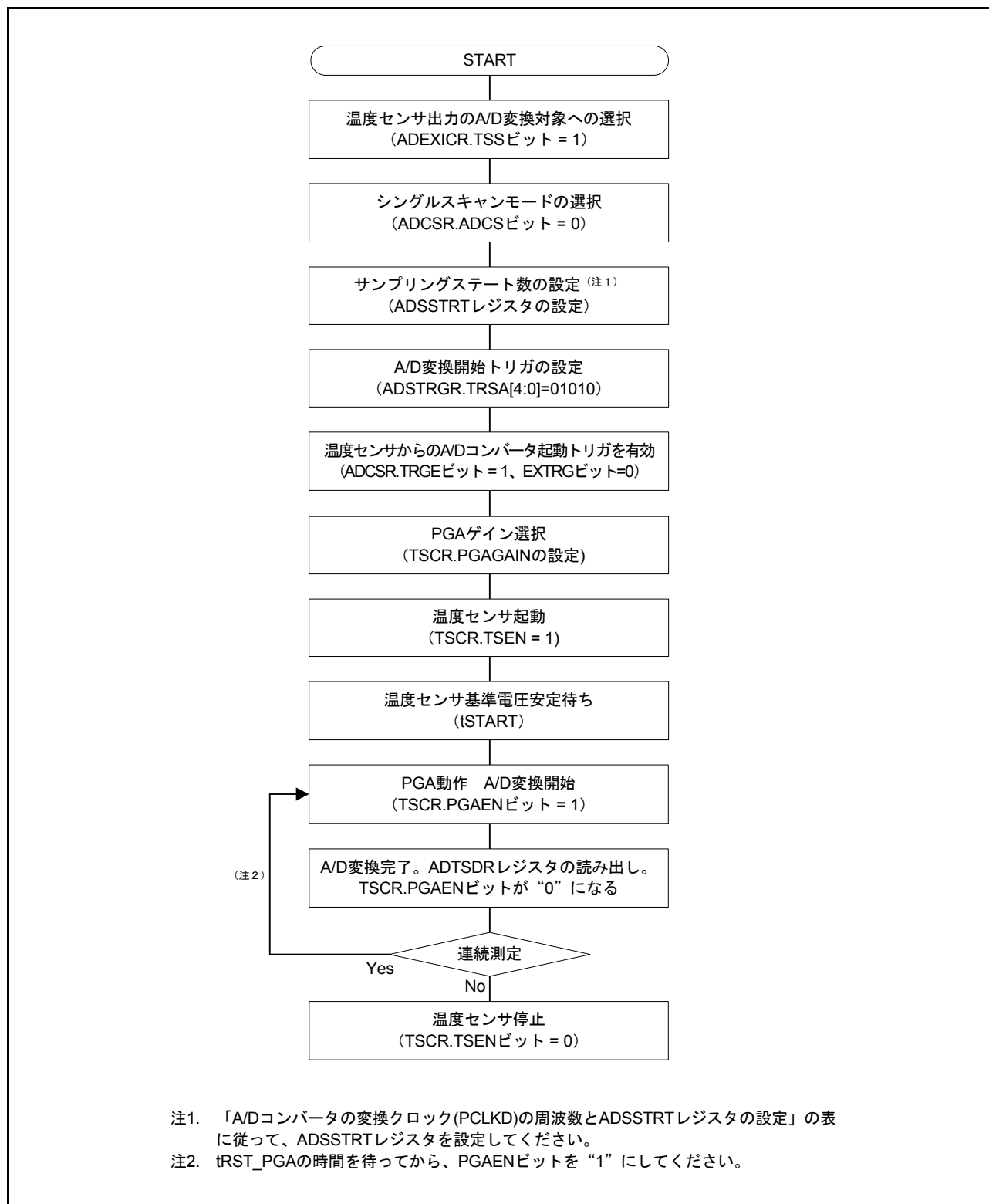
図 37.3 温度センサの使用手順フロー
