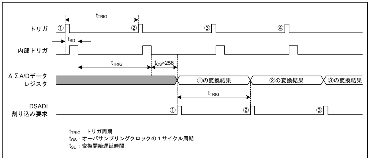
図 34.6 動作タイミングチャート
