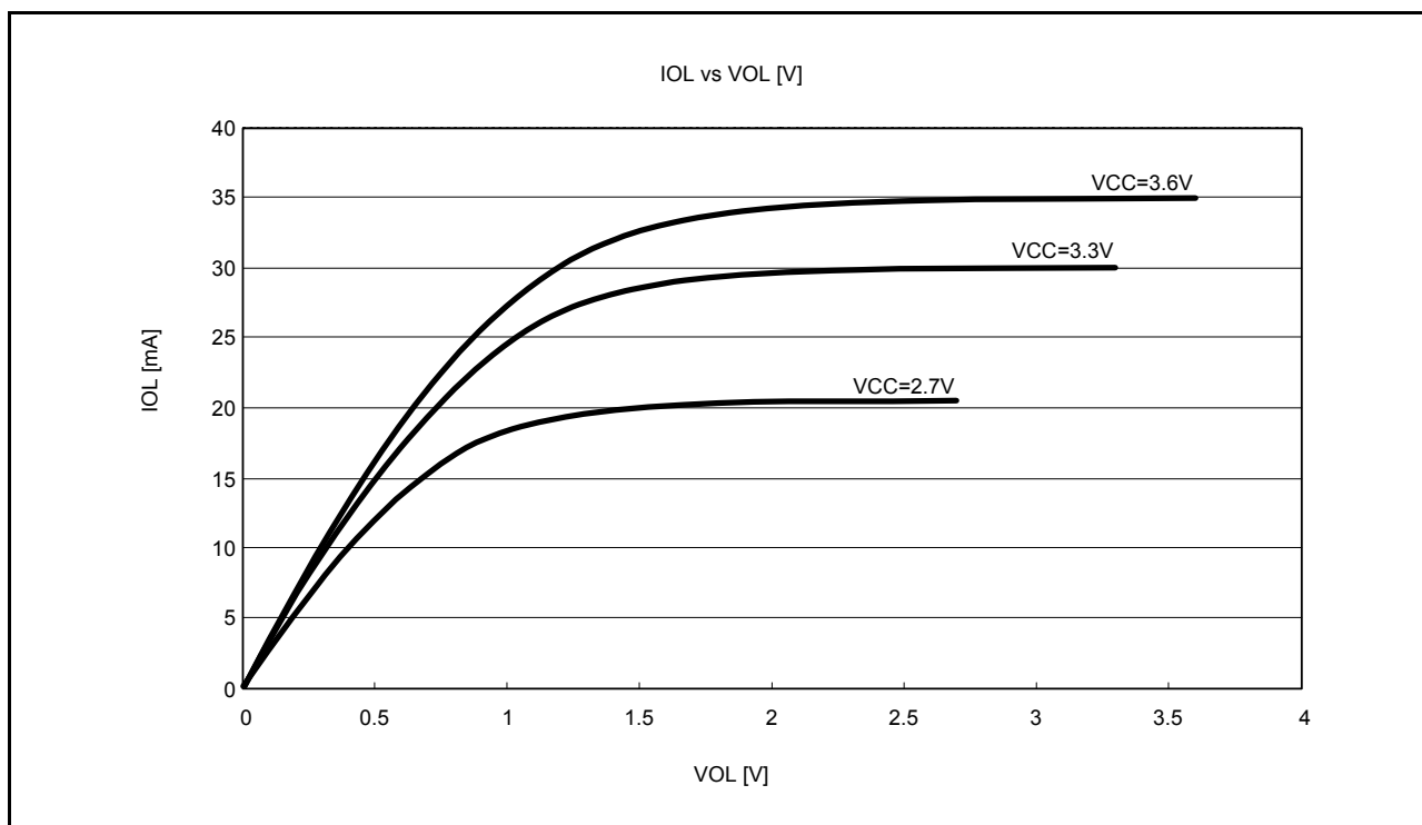
図 44.21 RIIC 出力端子の VOL、IOL 電圧特性 Ta = 25 °C (参考データ)
