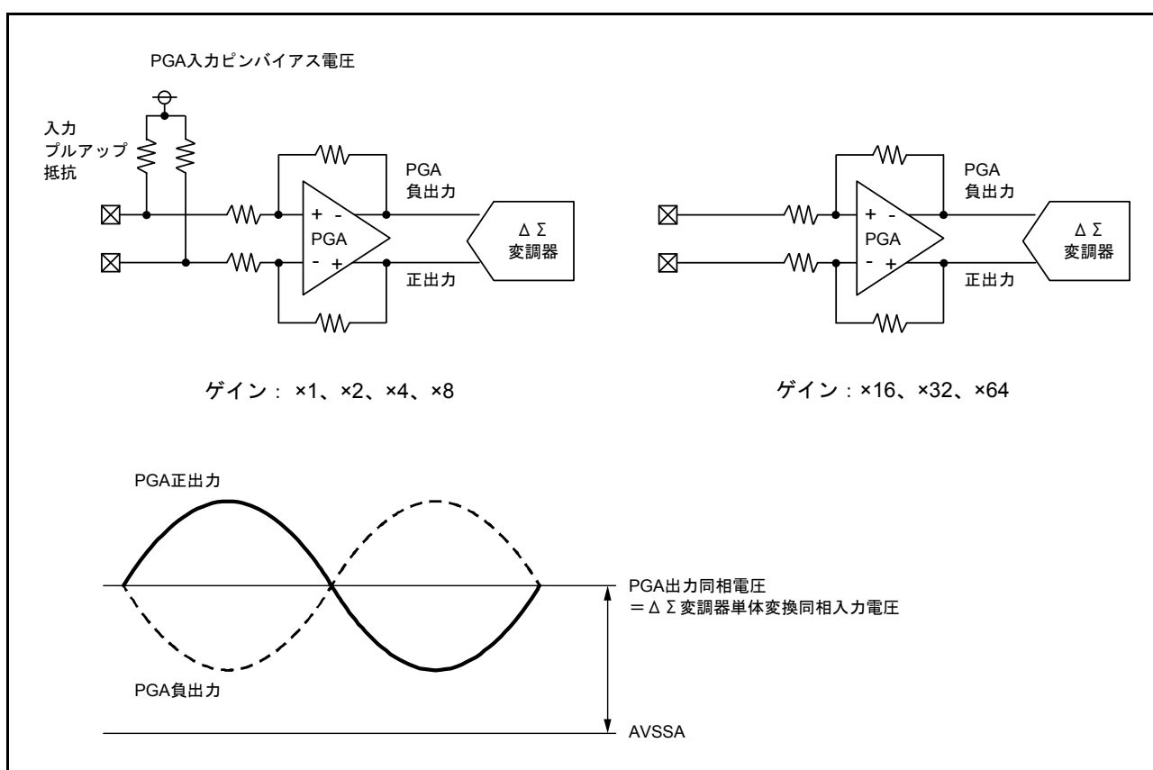
図 34.8 PGA 入力部のバイアス電圧印加
