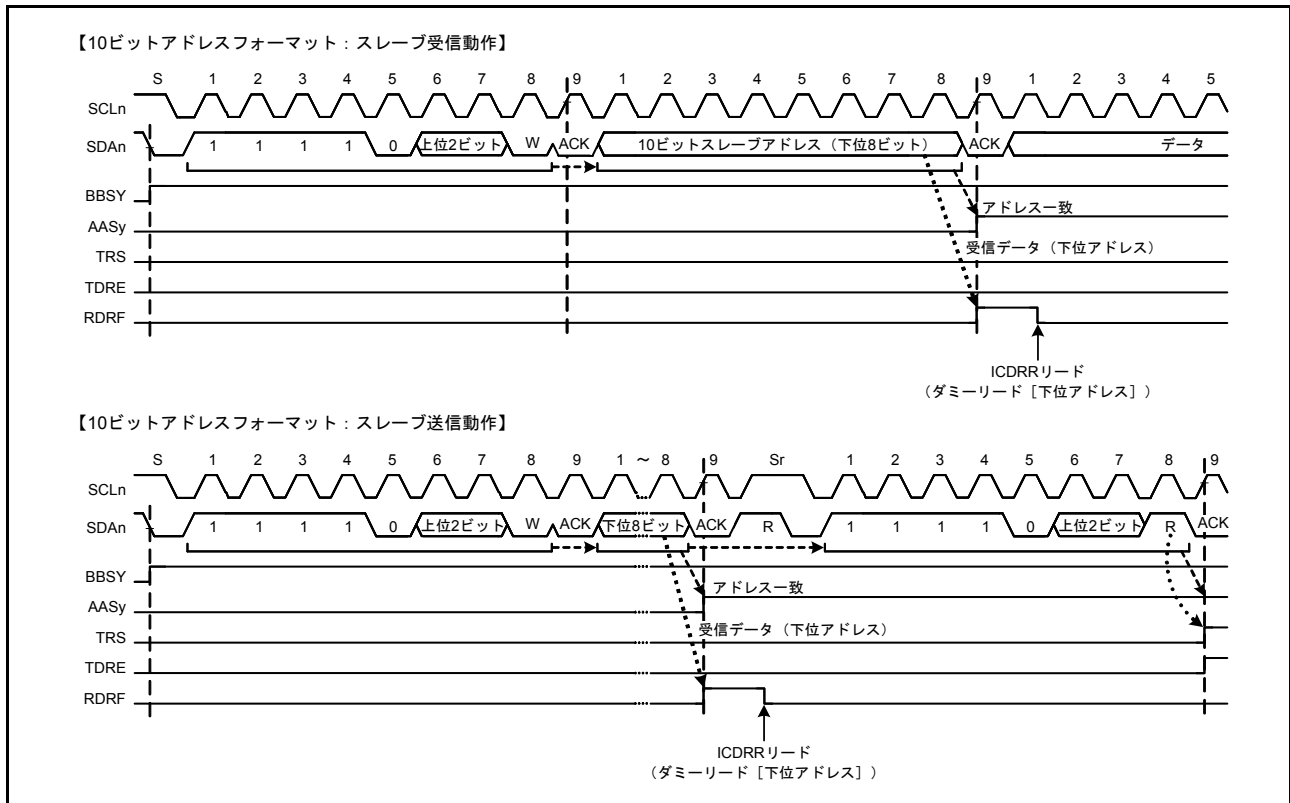
図 31.25 10ビットアドレスフォーマット選択時に AASy フラグが“1”になるタイミング
