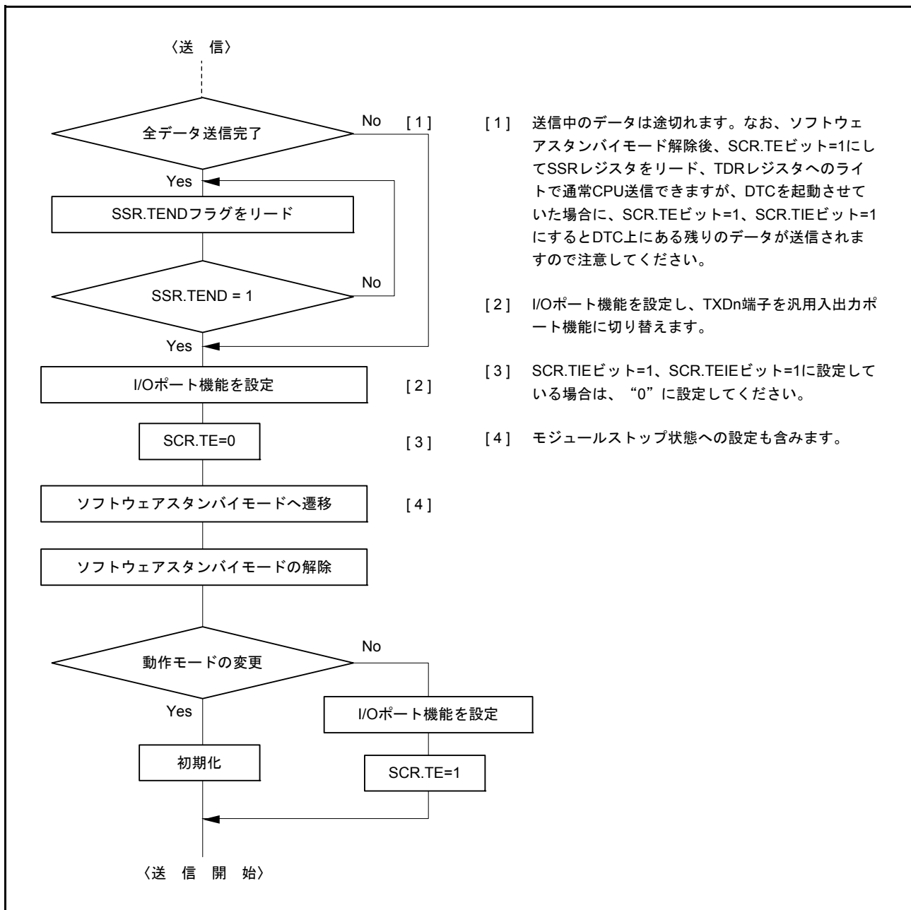
図 29.53 送信時のソフトウェアスタンバイモード遷移フローチャートの例
