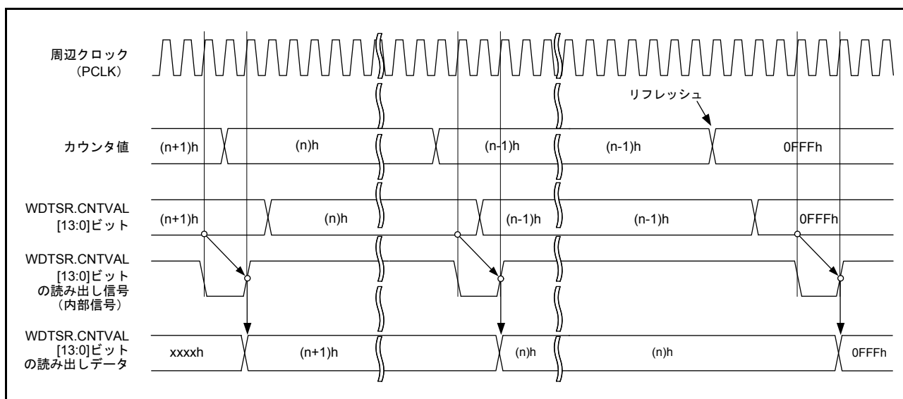
図 27.7 WDT ダウンカウンタ値の読み出し処理 (WDTCR.CKS[3:0] = 0100b、WDTCR.TOPS[1:0] = 01b)
