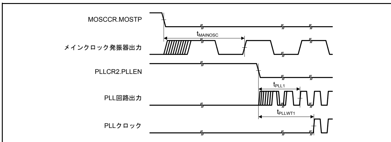
図 44.31 PLL クロック発振開始タイミング (メインクロック発振安定後に PLL を動作させたとき)
