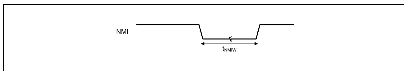
図 44.39 NMI 割り込み入カタイミング
