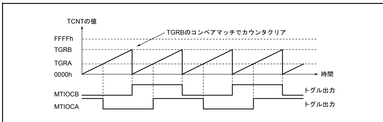
図 22.9 トグル出力の動作例
