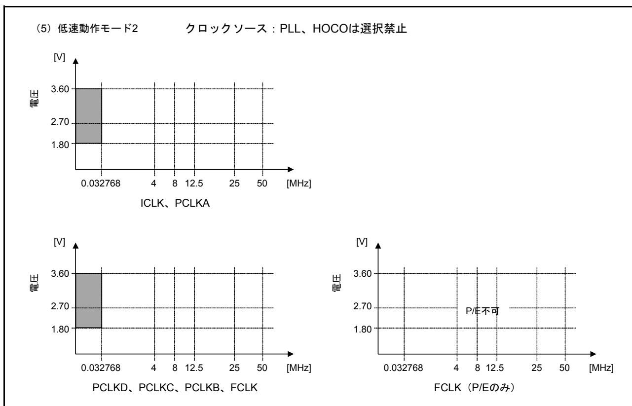
図 11.6 低速動作モード2 における動作電圧と動作周波数の関係
