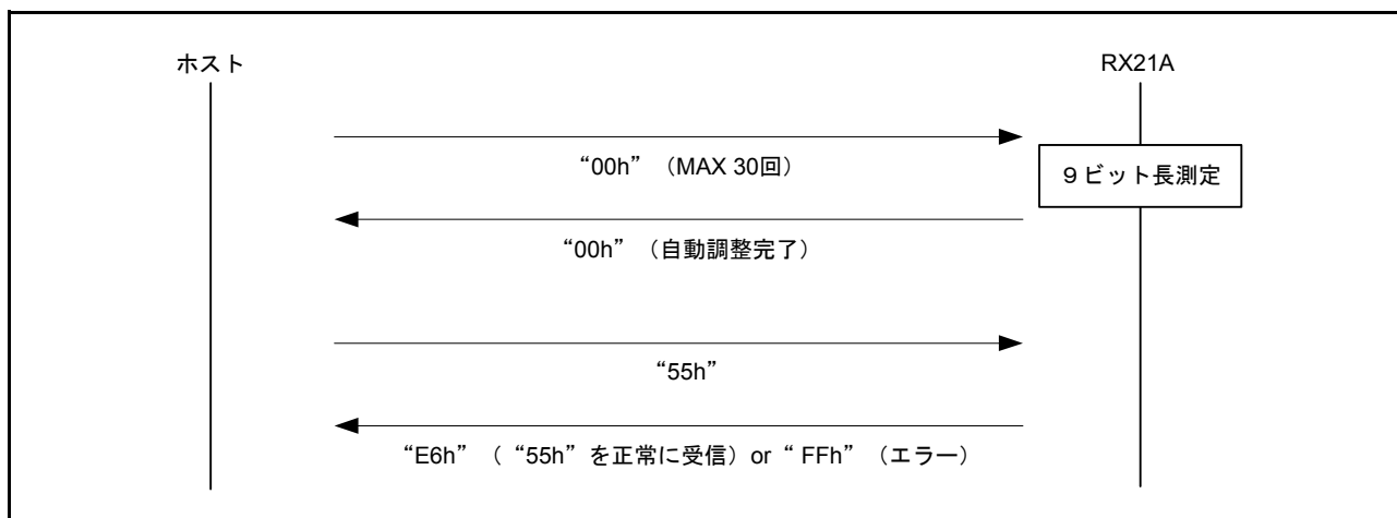
図 42.24 ホストと RX21A 間の通信シーケンス
