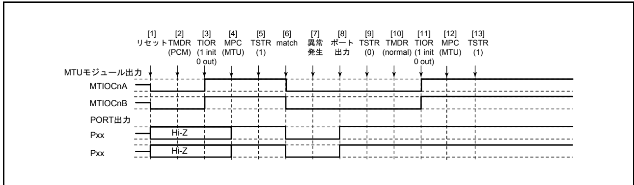
図 22.141 位相計数モードで異常が発生し、ノーマルモードで復帰する場合
