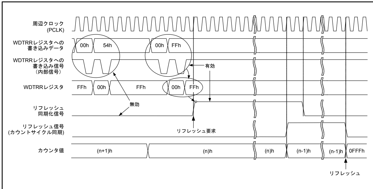
図 27.6 WDT リフレッシュ動作波形 (WDTCR.CKS[3:0] = 0100b、WDTCR.TOPS[1:0] = 01b)
