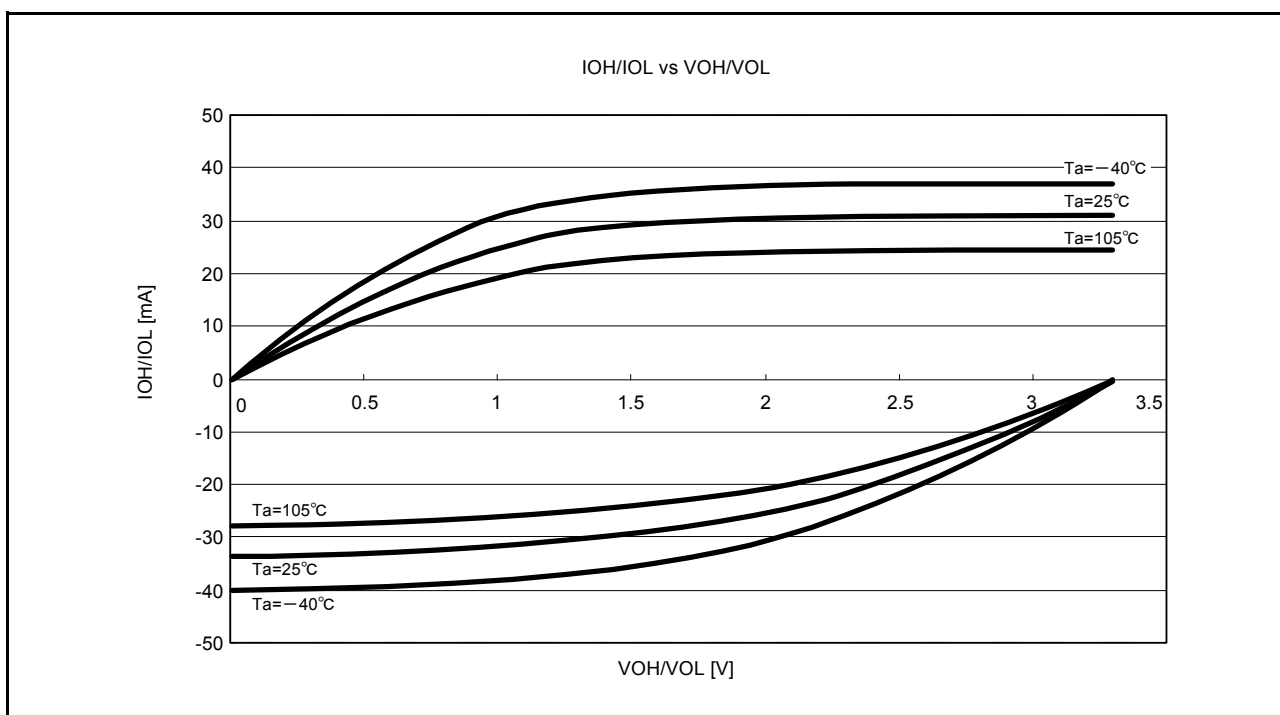
図 44.19 高駆動出力を選択したときの VOH/VOL IOH/IOL 温度特性 VCC = 3.3V (参考データ)
