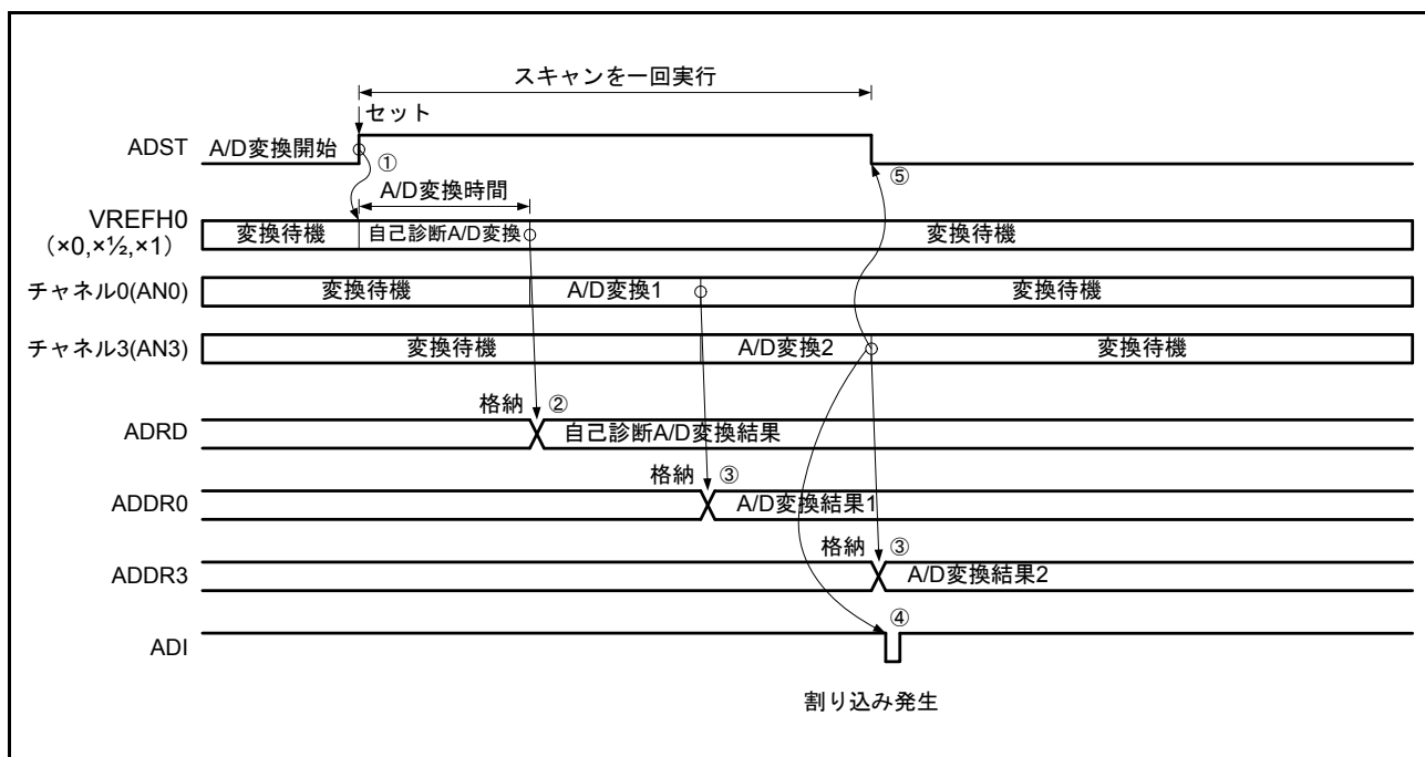
図 35.4 シングルスキャンモードの動作例 (基本動作+自己診断)
