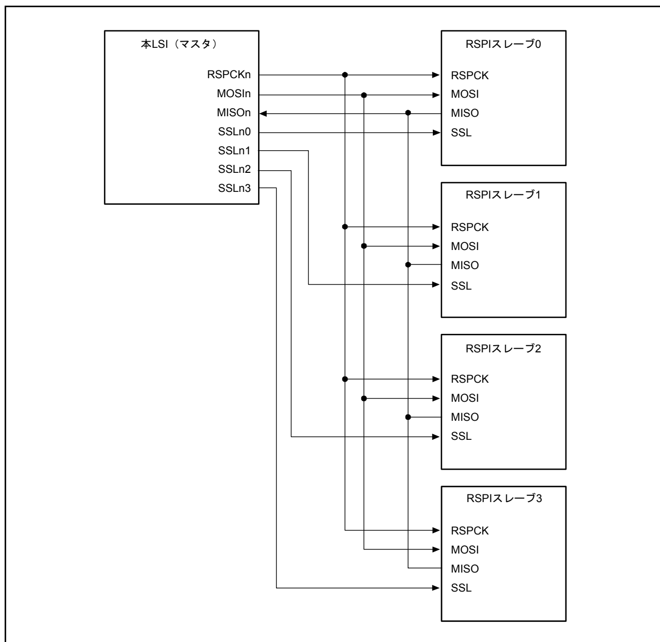
図 32.8 シングルマスタ / マルチスレーブの構成例 (本 LSI = マスタ)
