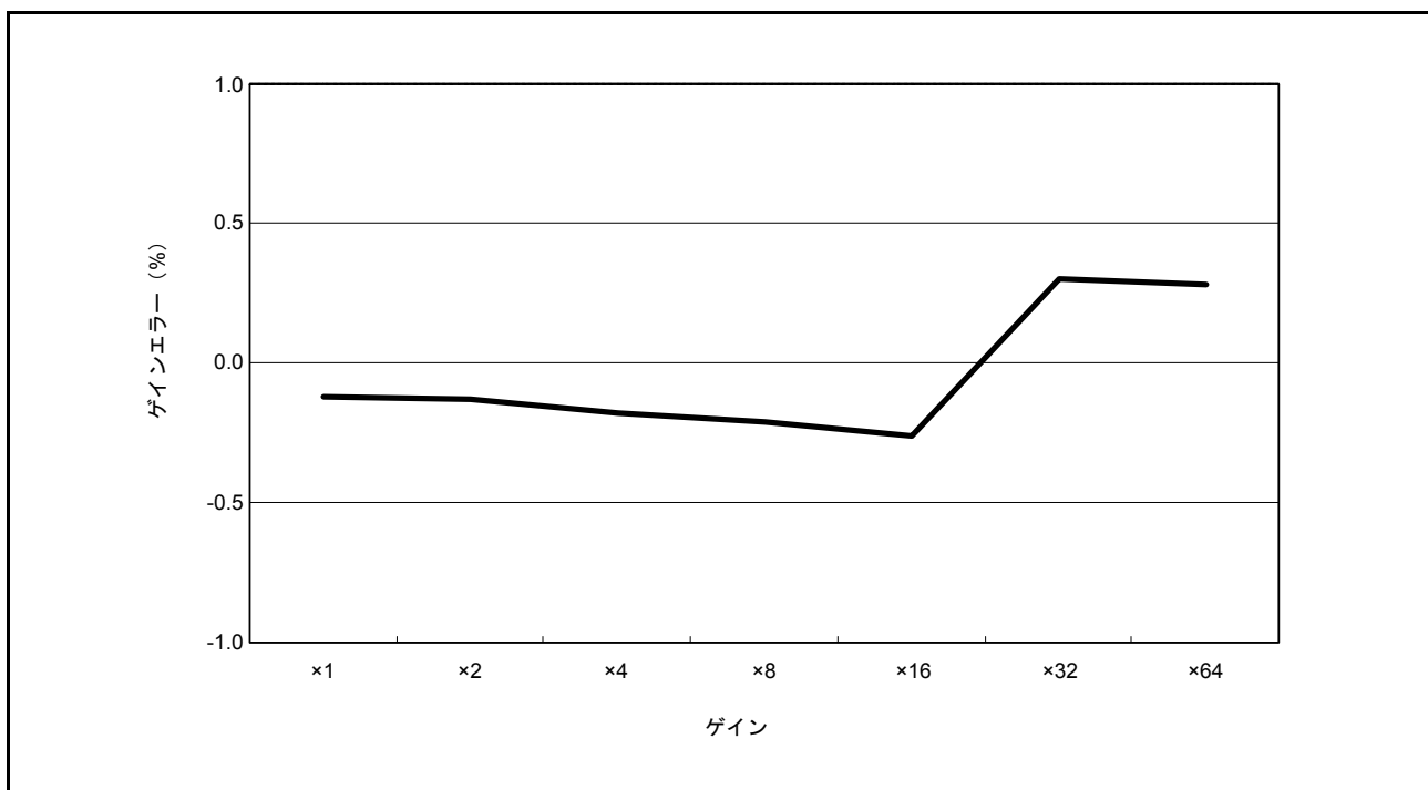
図 44.57 ゲインエラー (参考データ)
