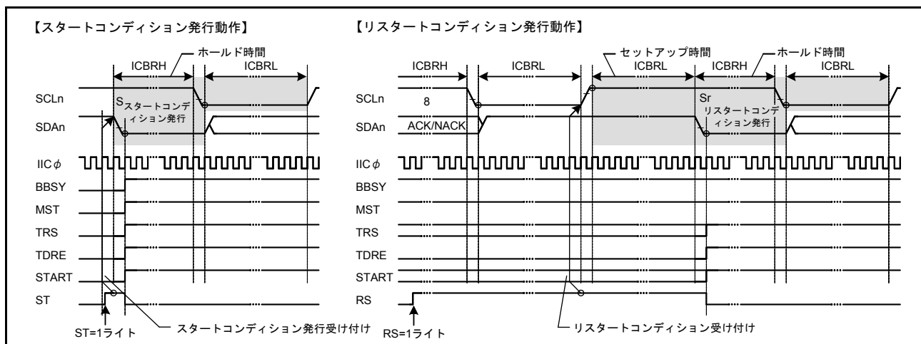
図 31.37 スタートコンディション/リスタートコンディション発行動作タイミング (ST、RS ビット)
