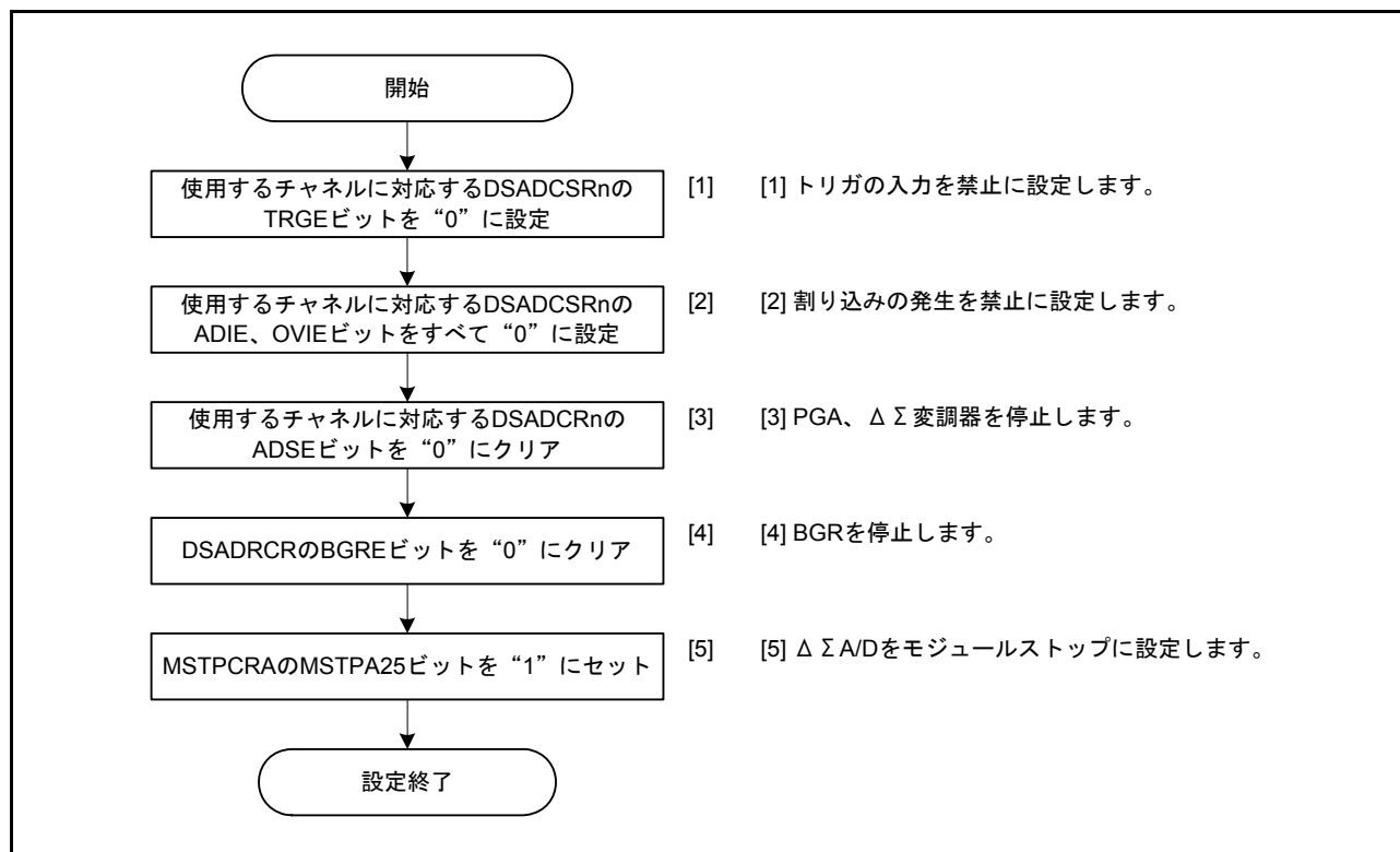
図 34.3 \Delta\Sigma A/Dコンバータの停止手順
