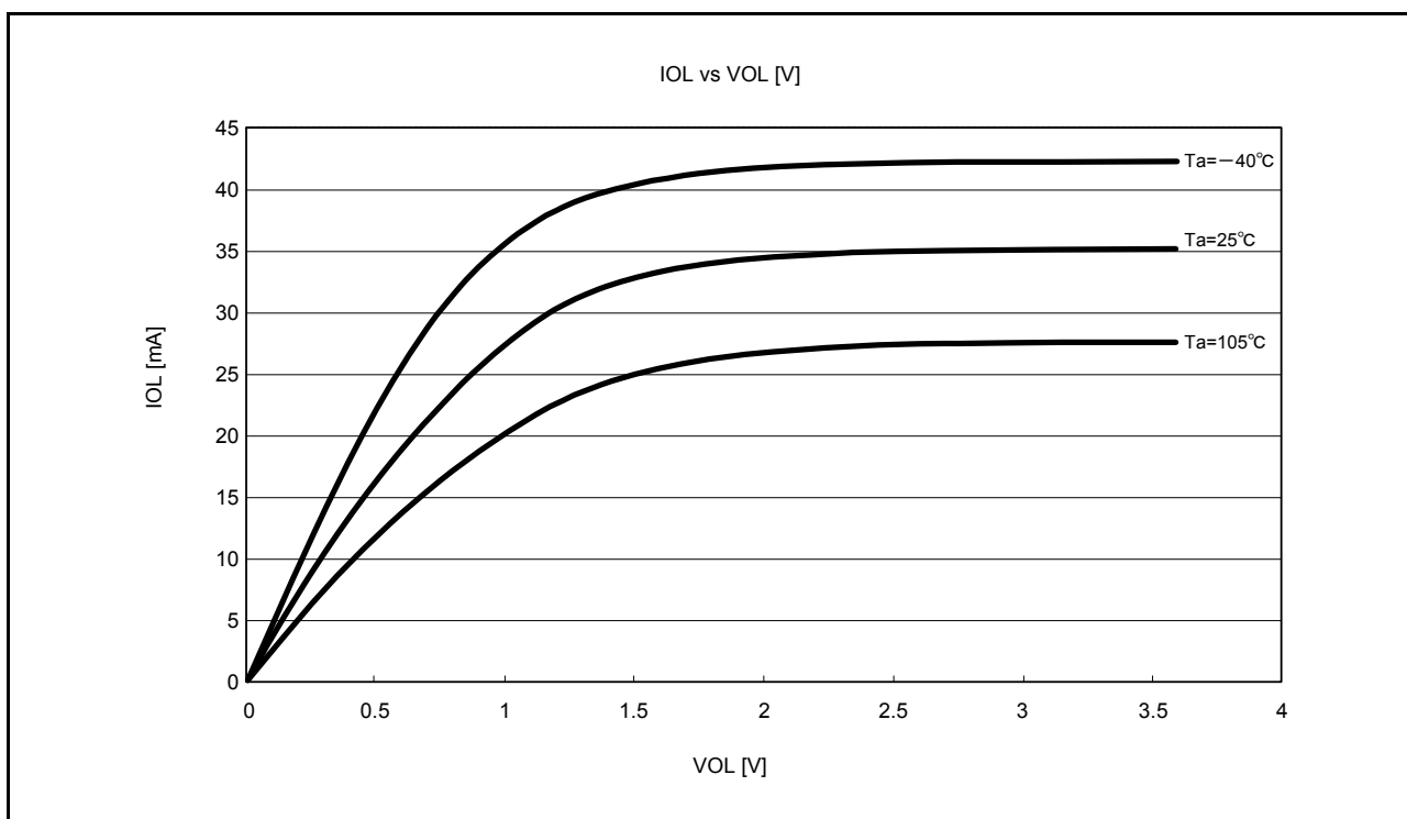
図 44.24 RIIC 出力端子の VOL、IOL 温度特性 VCC = 3.6V (参考データ)
