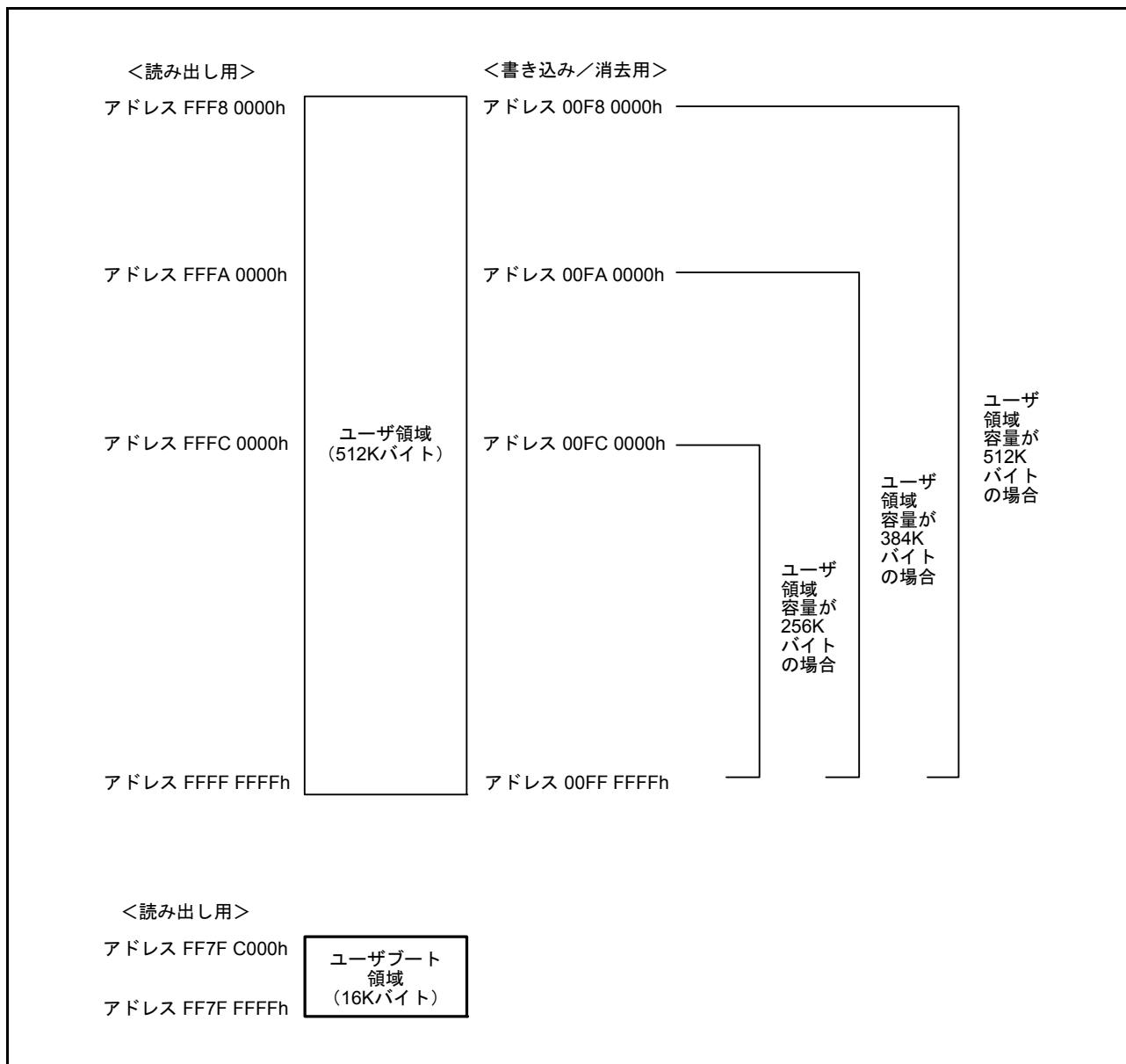
図 42.2 ROM の領域構成
