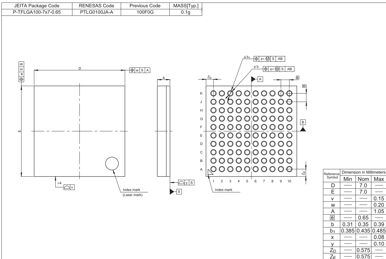
図 D. 100ピン TFLGA (PTLG0100JA-A)
