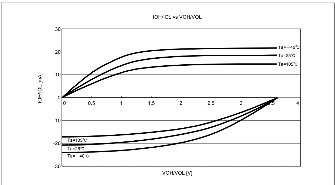
図 44.15 通常出力を選択したときの VOH/VOL IOH/IOL 温度特性 VCC = 3.6V (参考データ)
