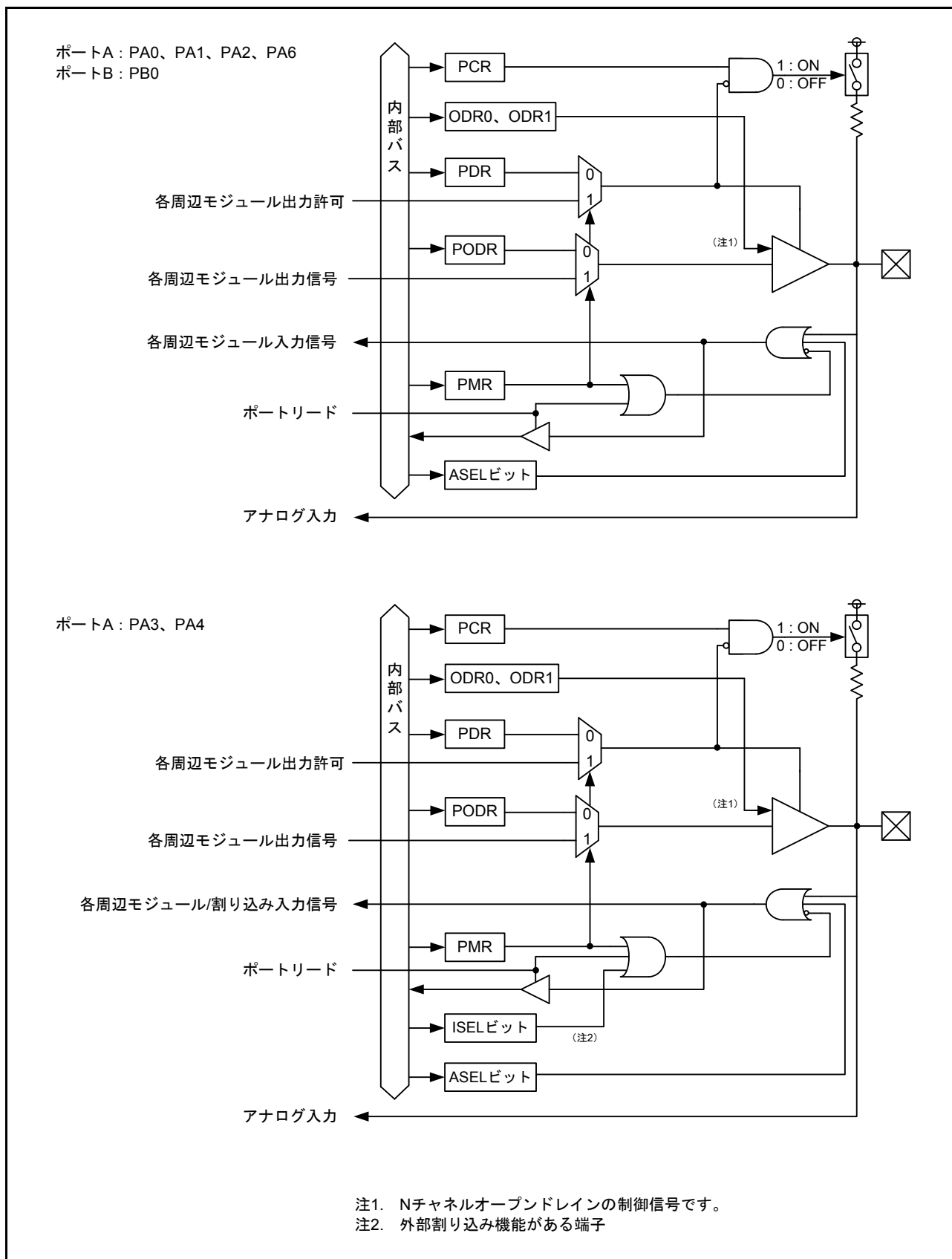
図 20.4 入出力ポートの構成 (4)
