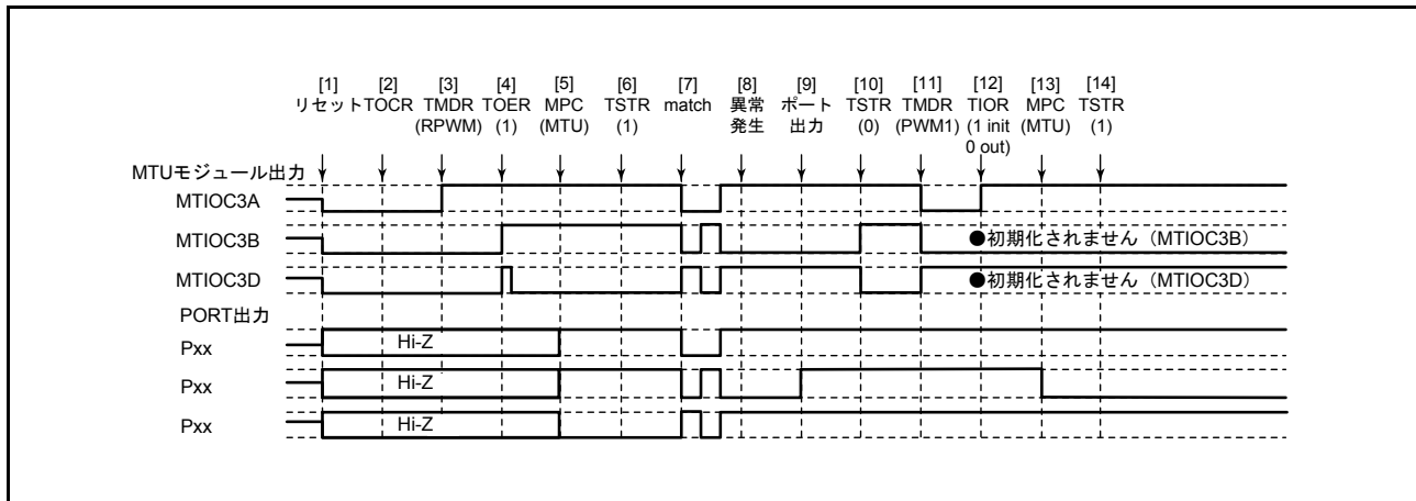
図 22.151 リセット同期 PWM モードで異常が発生し、PWM モード 1 で復帰する場合
