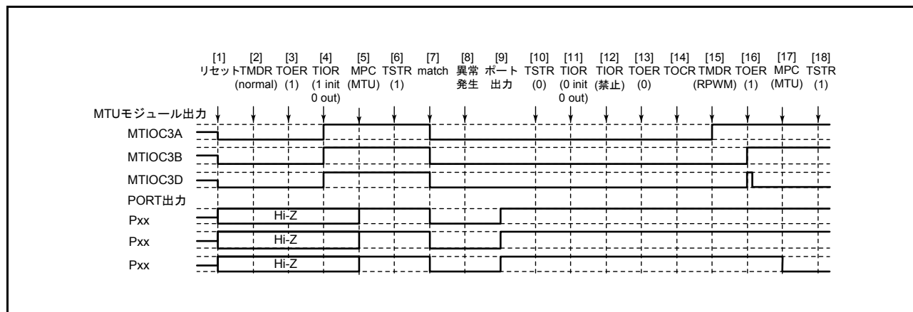
図 22.130 ノーマルモードで異常が発生し、リセット同期 PWM モードで復帰する場合
