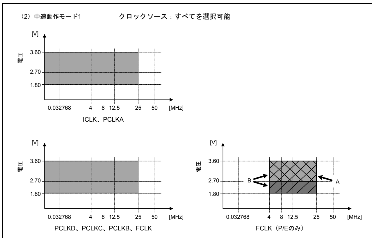
図 11.3 中速動作モード 1A、1B における動作電圧と動作周波数の関係
