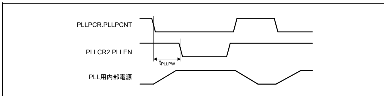
図 44.33 PLL 電源制御タイミング
