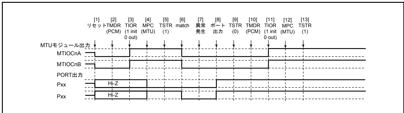
図 22.144 位相計数モードで異常が発生し、位相計数モードで復帰する場合
