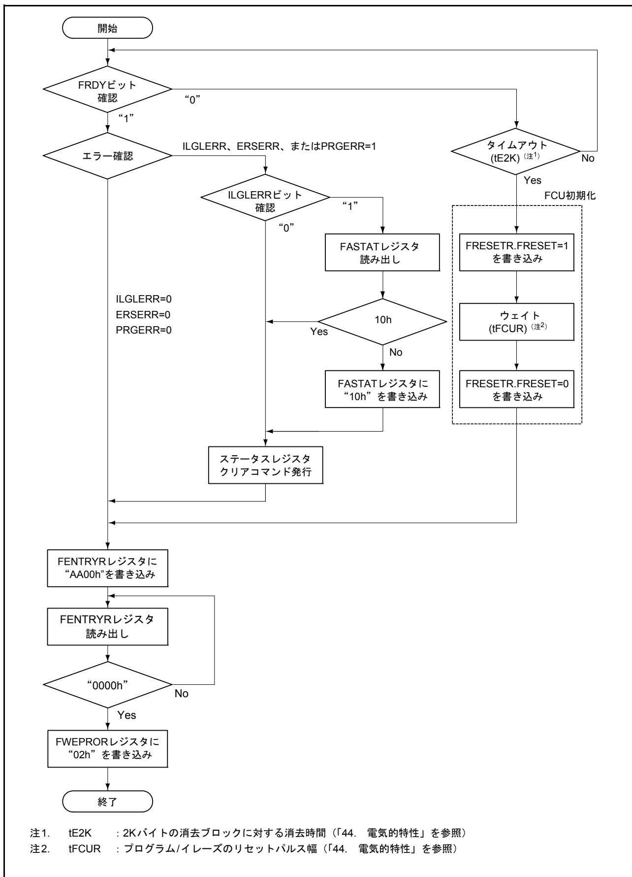
図 42.6 ROM リードモード移行フロー
