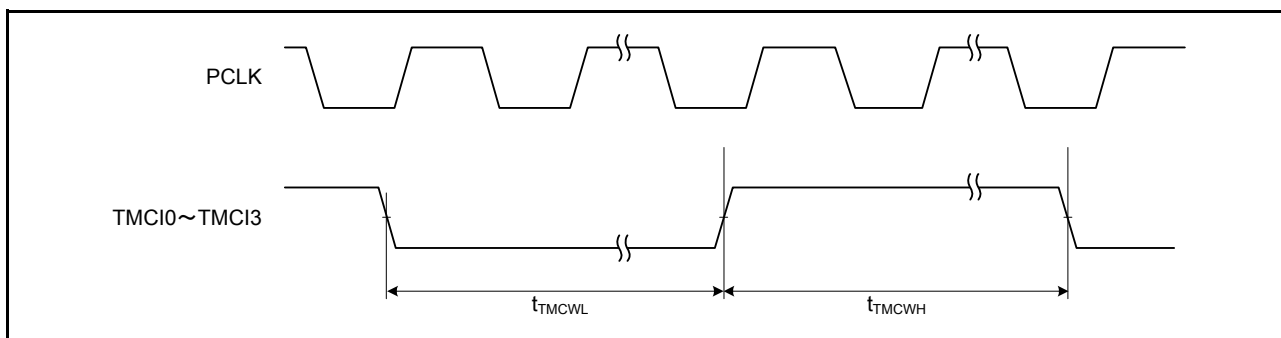
図 44.45 8ビットタイマクロック入力タイミング
