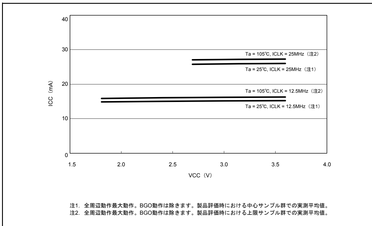
図 44.3 中速動作モード 2A、2B の電圧依存性 (参考データ)
