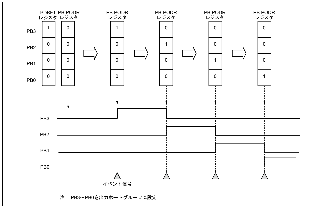
図 19.6 出力ポートグループのビットローテート動作
