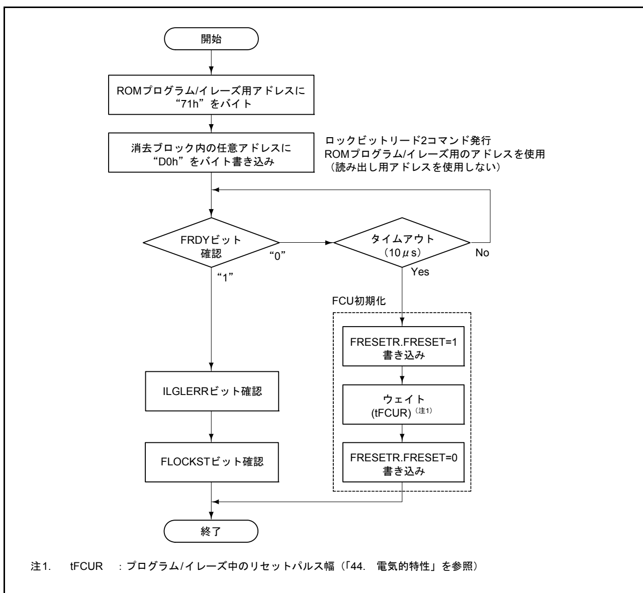
図 42.15 レジスタリード方式でロックビットを読み出す方法
