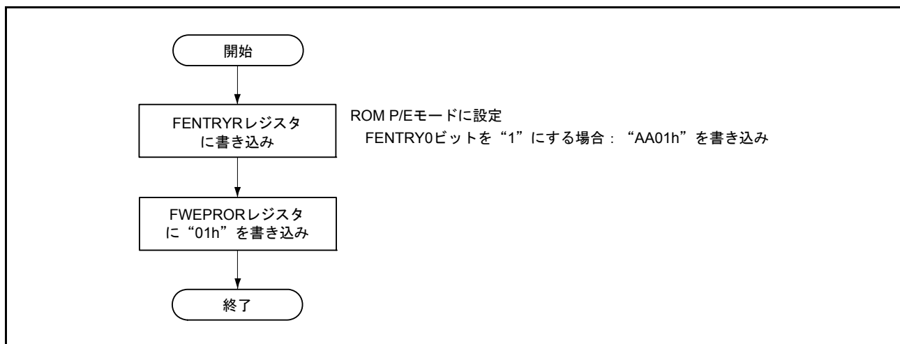
図 42.5 ROM P/E モード移行フロー
