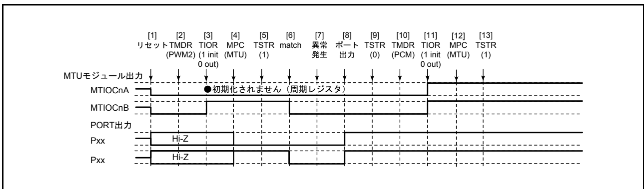
図 22.140 PWM モード 2 で異常が発生し、位相計数モードで復帰する場合
