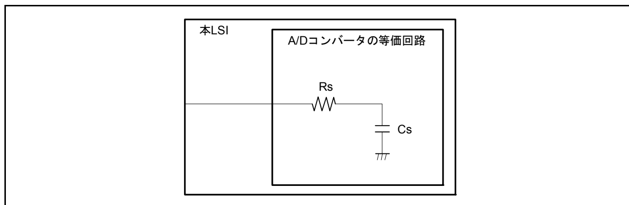
図 35.17 アナログ入力端子の内部等価回路
