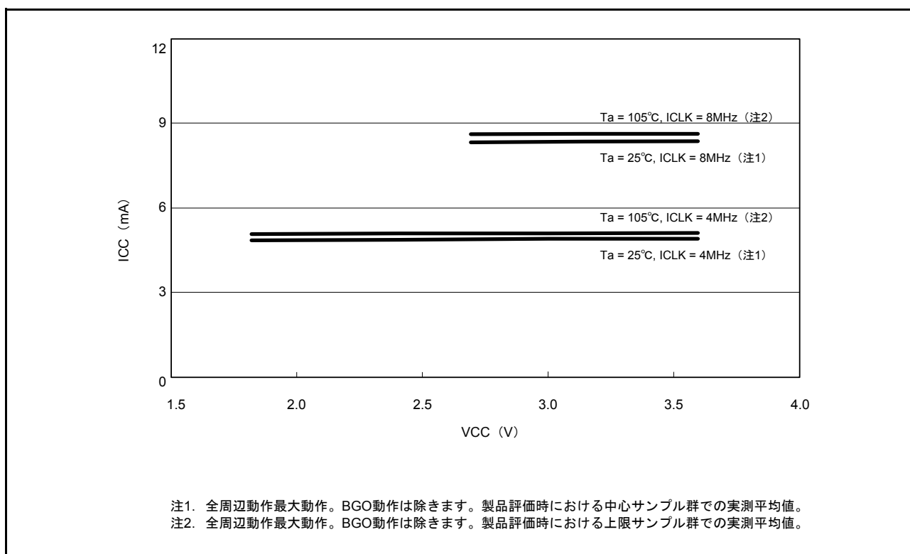
図 44.4 低速動作モード 1 の電圧依存性 (参考データ)
