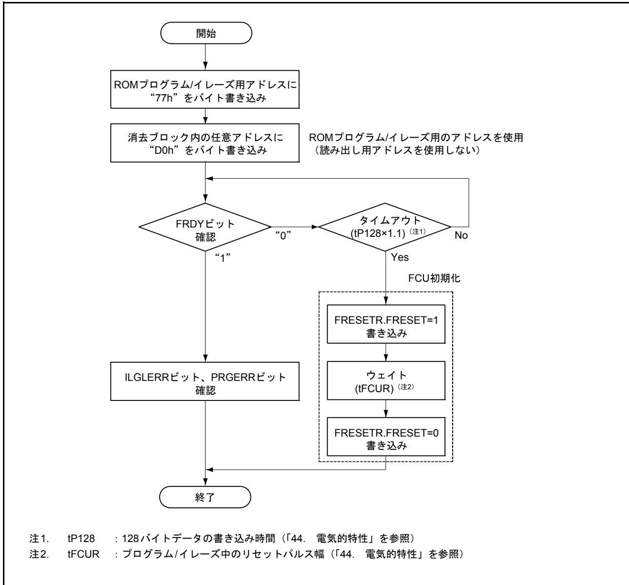
図 42.14 ロックビットのプログラムの設定方法
