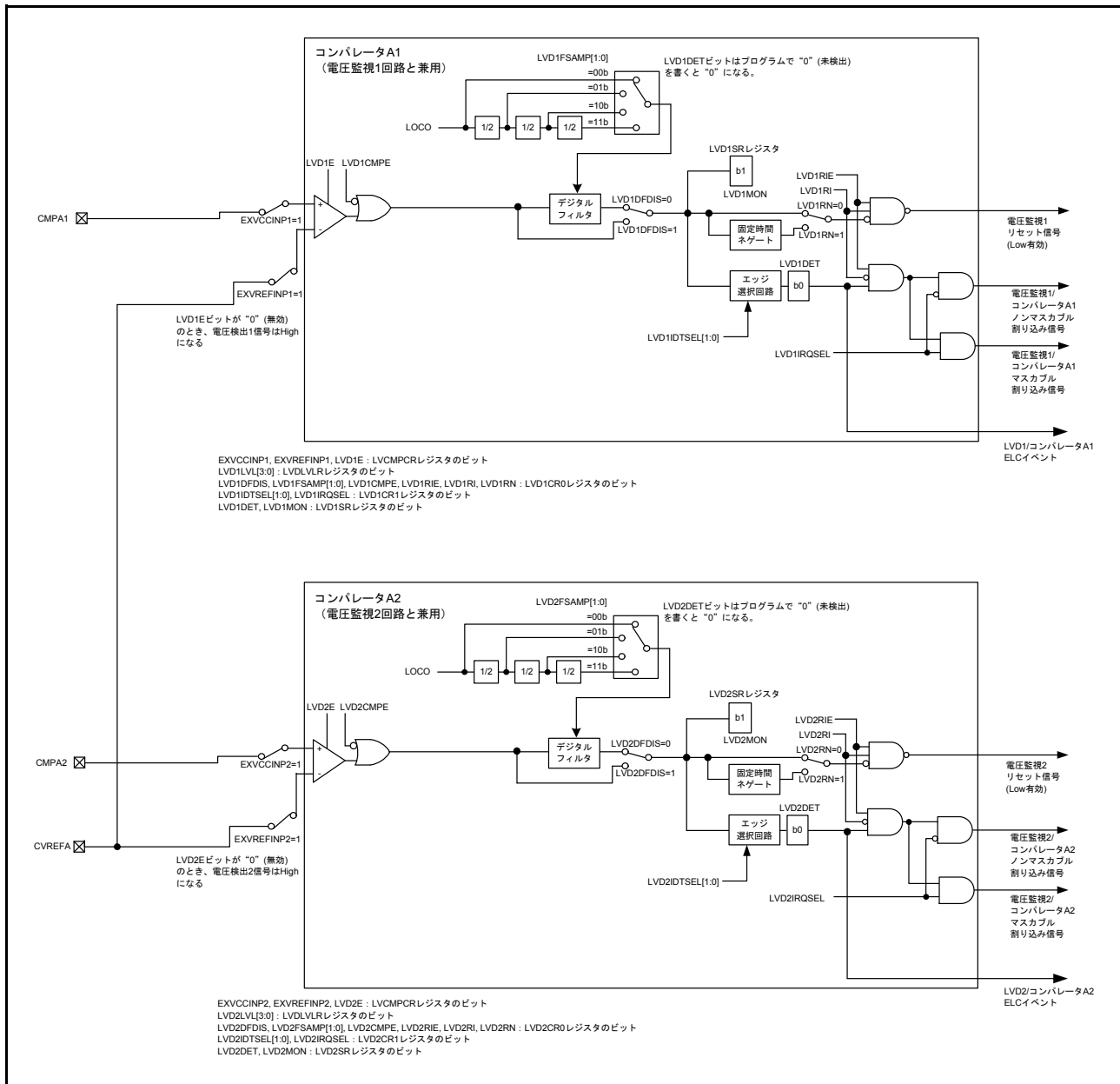
図 38.1 コンパレータ A のブロック図
