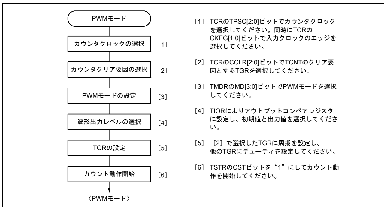
図 22.25 PWM モードの設定手順例
