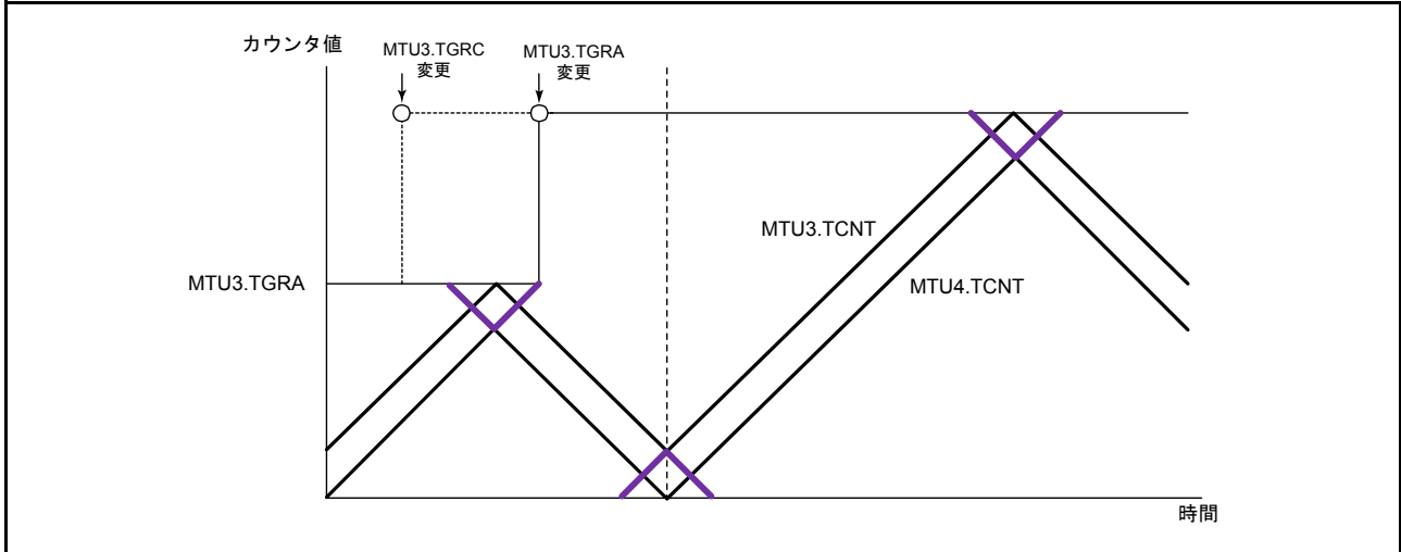
図 22.42 PWM 周期の変更例
