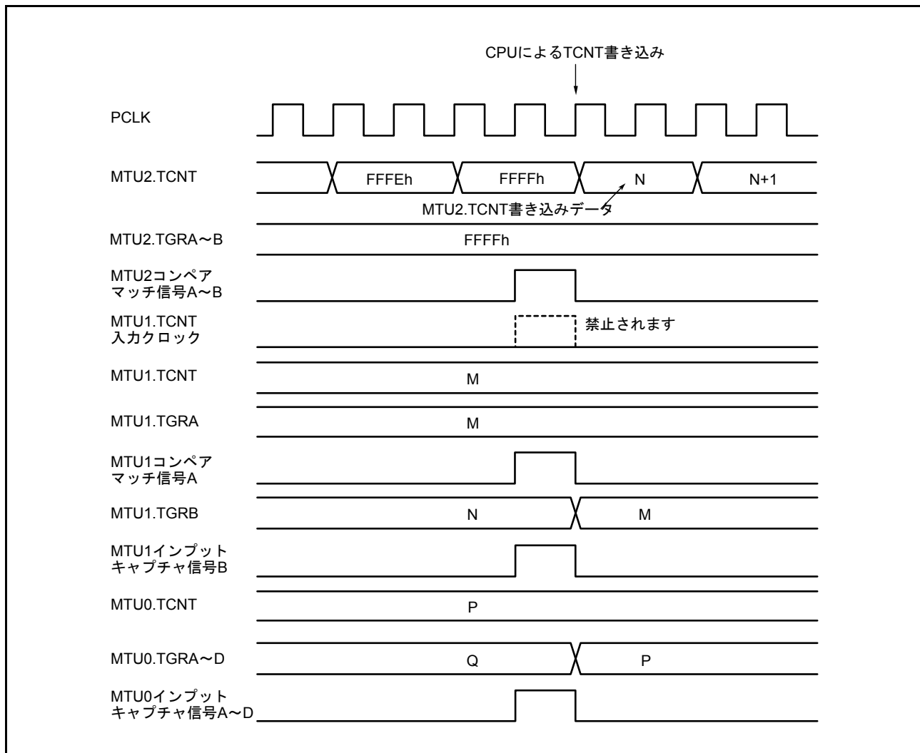
図 22.116 カスケード接続における MTU2.TCNT の書き込みとオーバーフロー/アンダフローの競合
