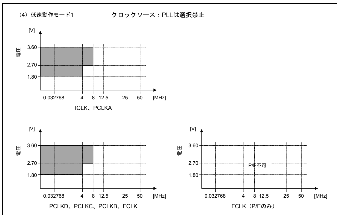
図 11.5 低速動作モード1における動作電圧と動作周波数の関係
