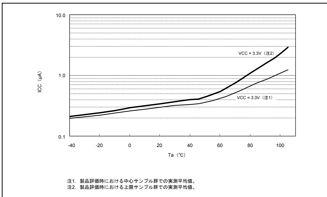
図 44.9 ディープソフトウェアスタンバイモード (DEEPCUT1 ビット = 1) 時の温度依存性 (参考データ)
