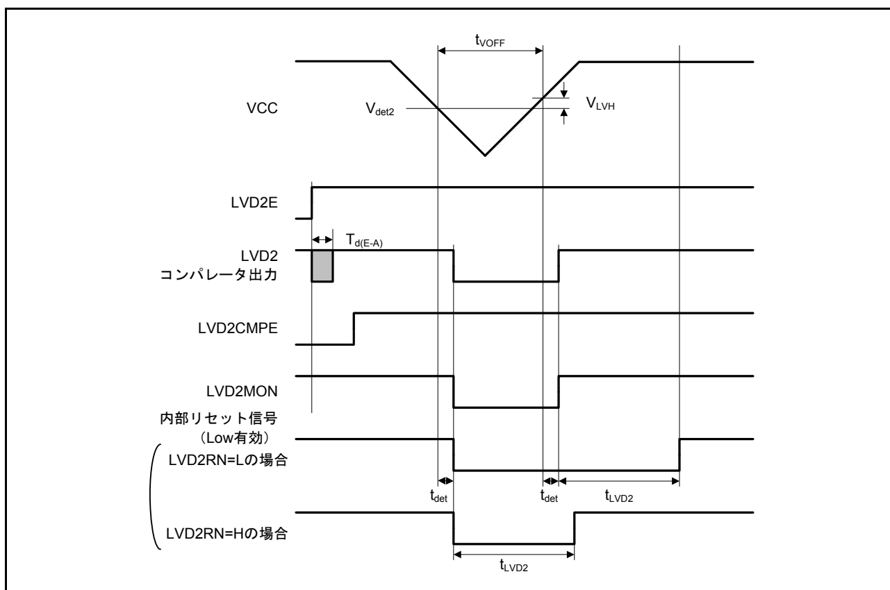
図 44.68 電圧検出回路タイミング (V det2 )
