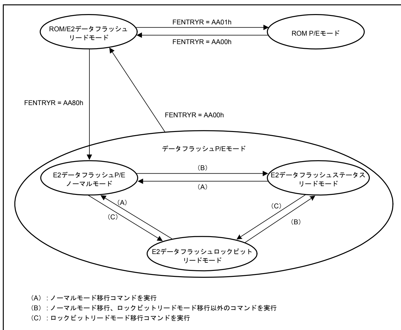
図 43.4 FCUのモード遷移図（E2データフラッシュ関連）
