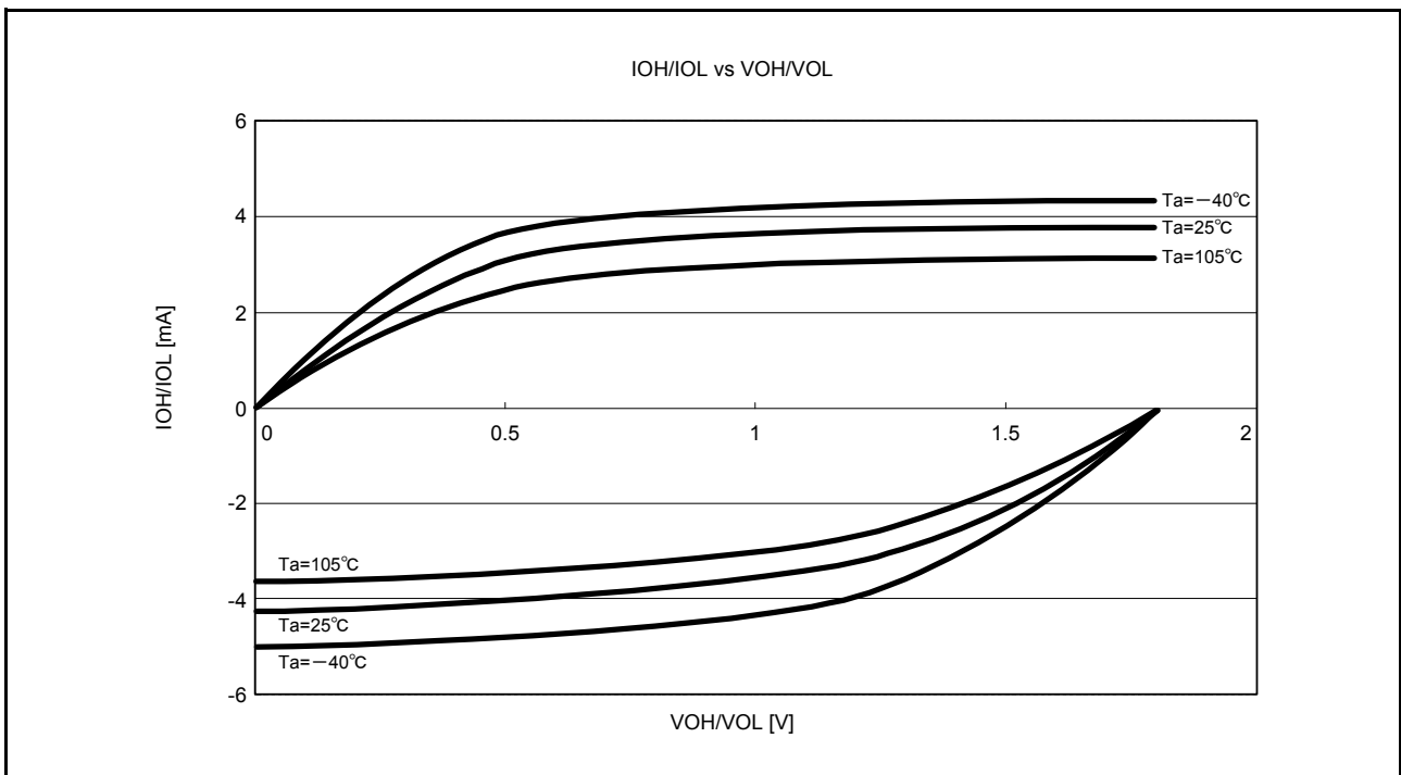
図 44.12 通常出力を選択したときの VOH/VOL IOH/IOL 温度特性 VCC = 1.8V (参考データ)
