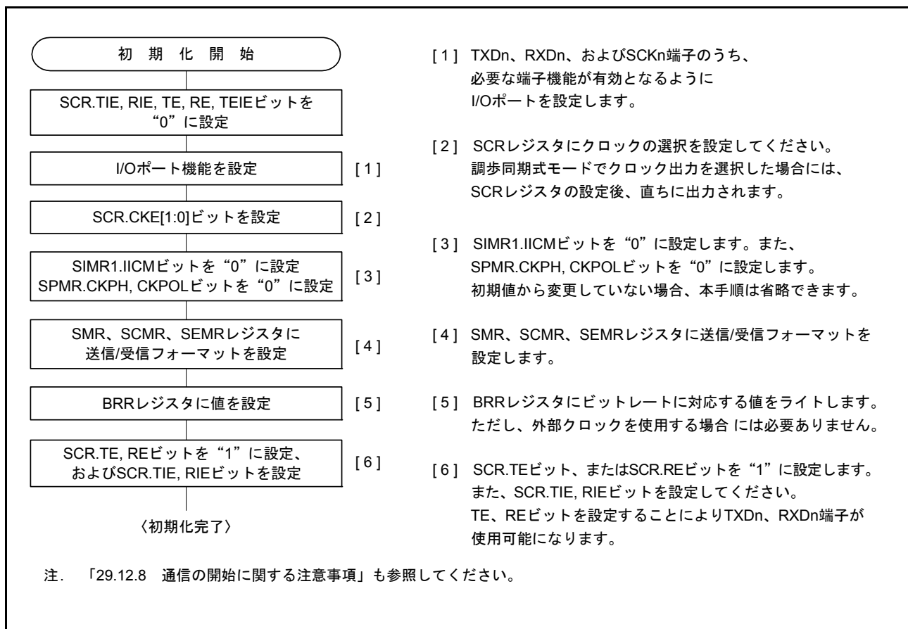
図 29.7 SCIの初期化フローチャートの例（調歩同期式モード）
