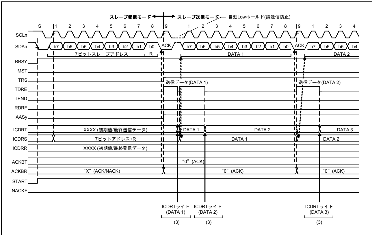
図 31.16 スレーブ送信の動作タイミング (1) (7ビットアドレスフォーマットの時)
