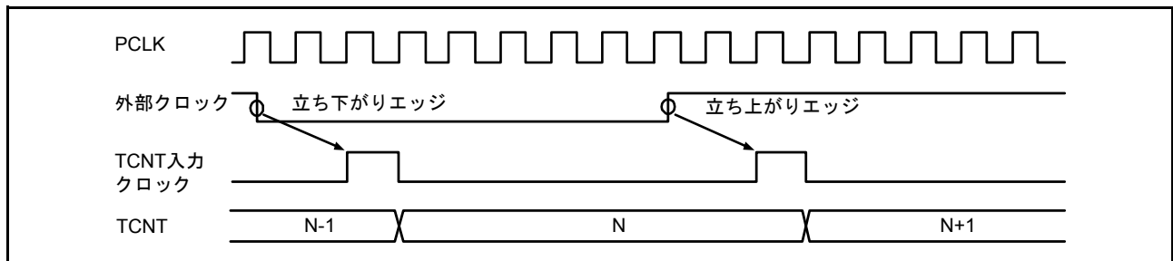
図 22.86 外部クロック動作時のカウントタイミング (MTU0 ~ MTU4)
