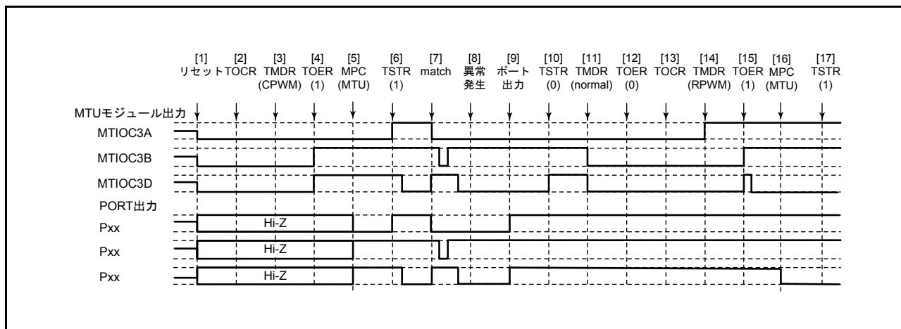
図 22.149 相補 PWM モードで異常が発生し、リセット同期 PWM モードで復帰する場合
