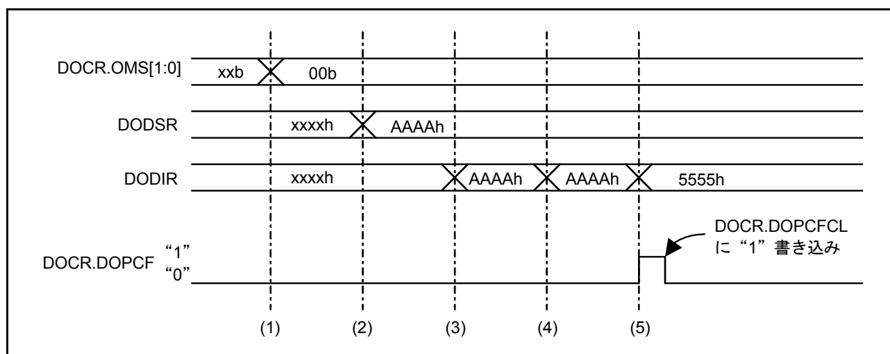
図 40.2 データ比較モードの動作例
