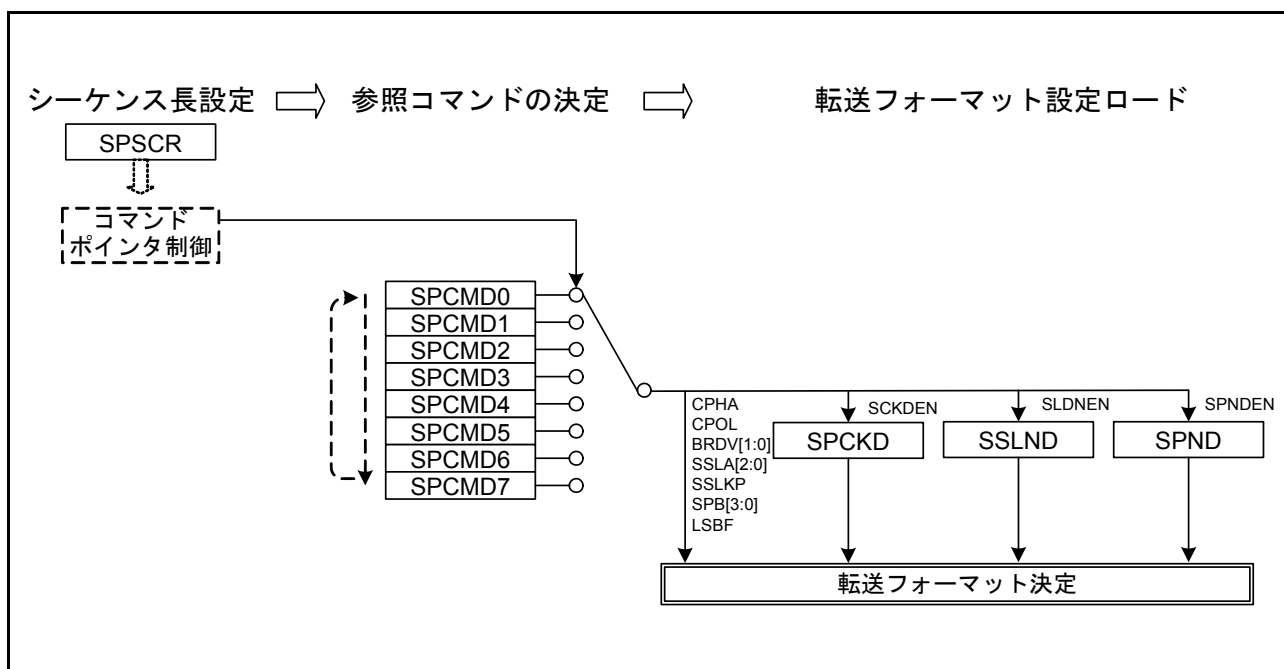
図 32.42 マスタモードでのシリアル転送方式の決定方法
