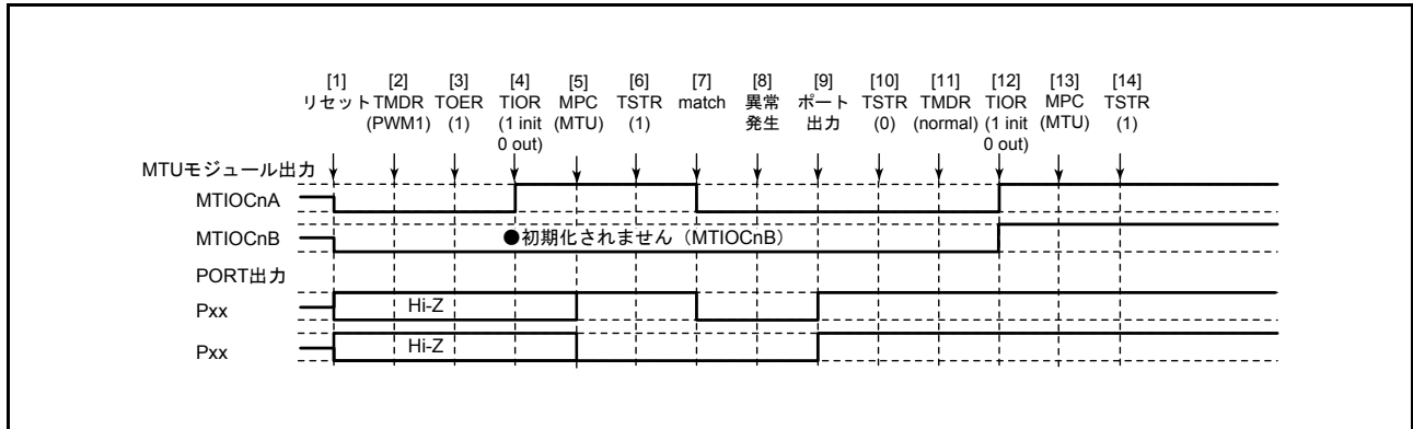
図 22.131 PWM モード 1 で異常が発生し、ノーマルモードで復帰する場合
