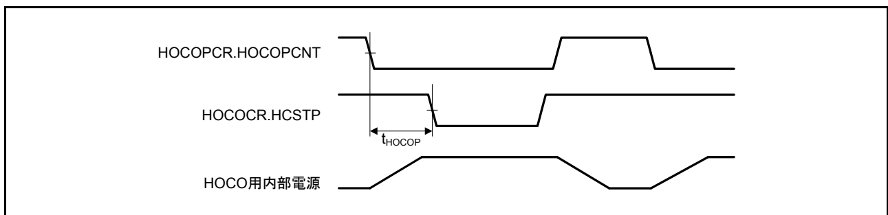
図 44.30 HOCO 電源制御タイミング
