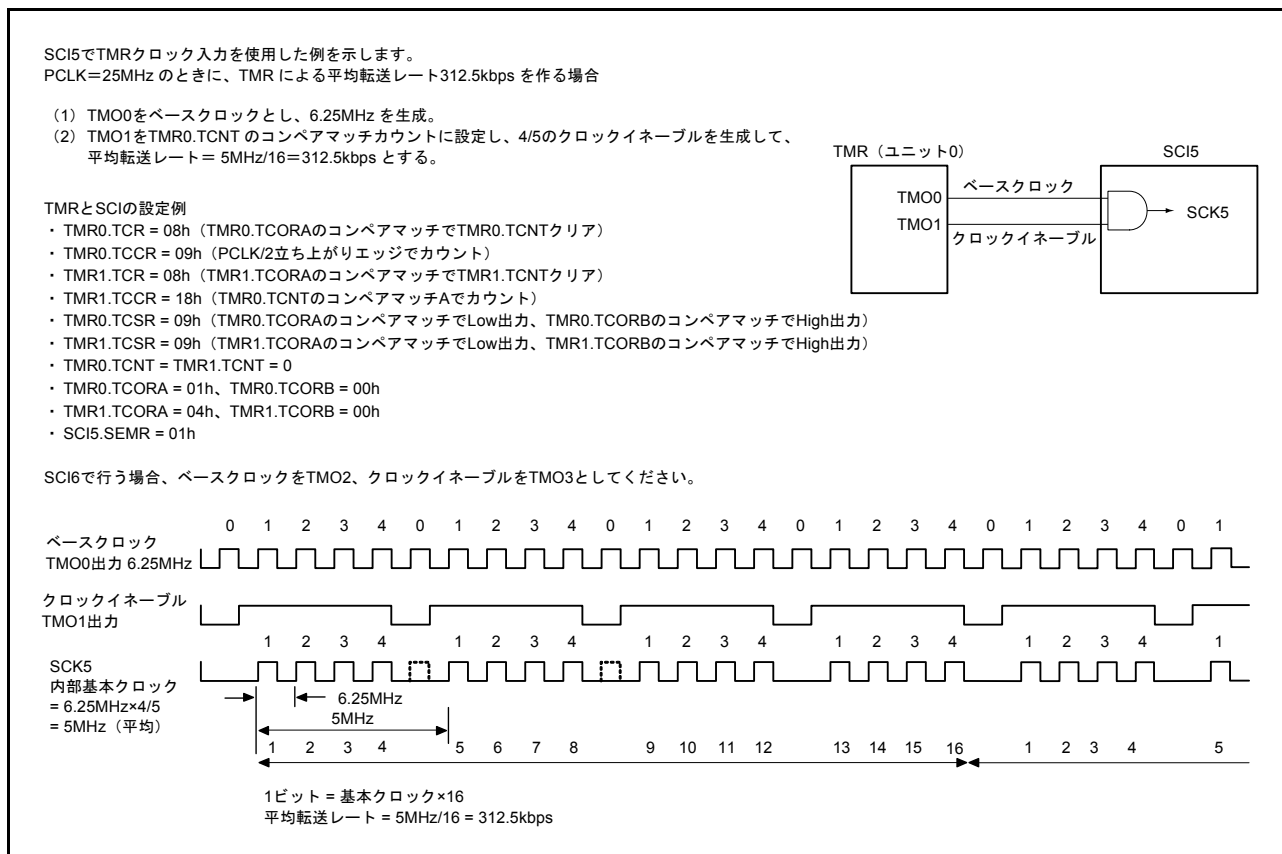
図 29.3 TMR クロック入力時の平均転送レート設定例
