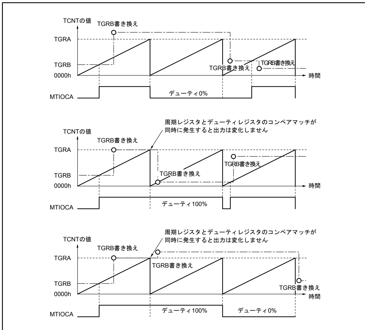
図 22.28 PWM モード動作例
