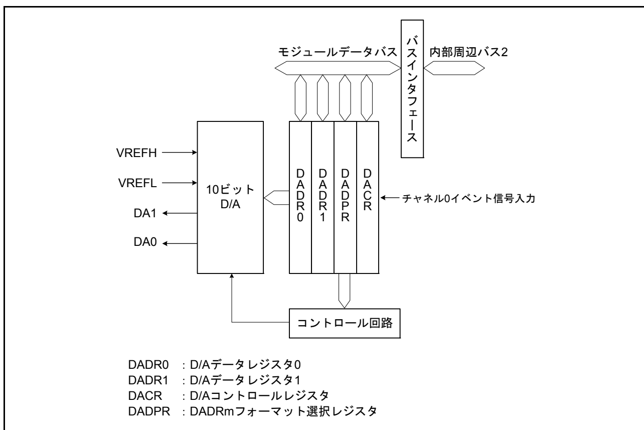
図 36.1 D/Aコンバータのブロック図
