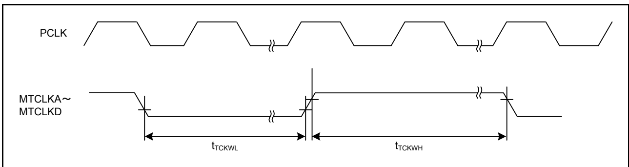
図 44.43 MTU クロック入力タイミング
