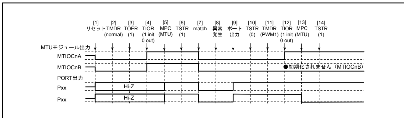
図 22.126 ノーマルモードで異常が発生し、PWM モード 1 で復帰する場合
