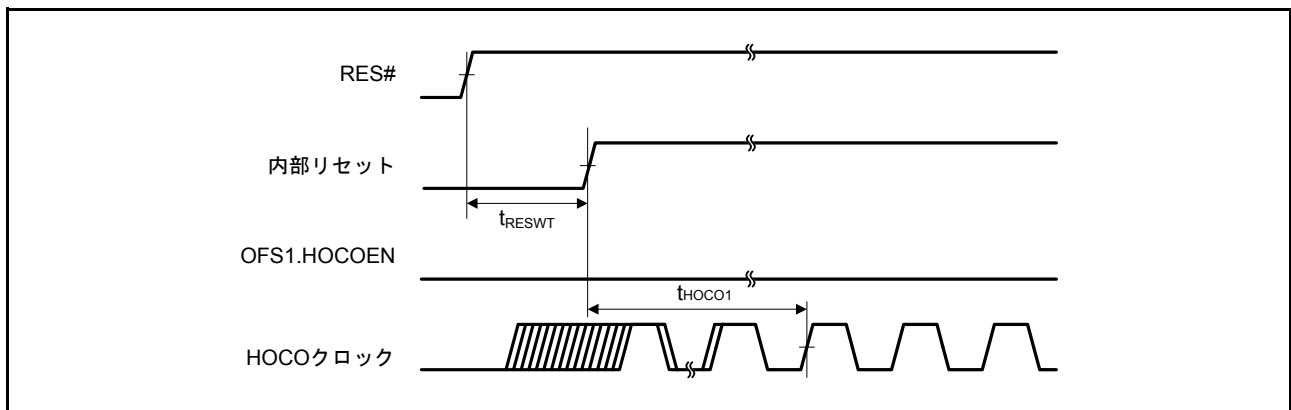
図 44.28 HOCO クロック発振開始タイミング (OFS1.HOCOEN ビット“0” 設定時のリセット解除後)
