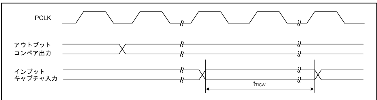
図 44.42 MTU 入出力タイミング
