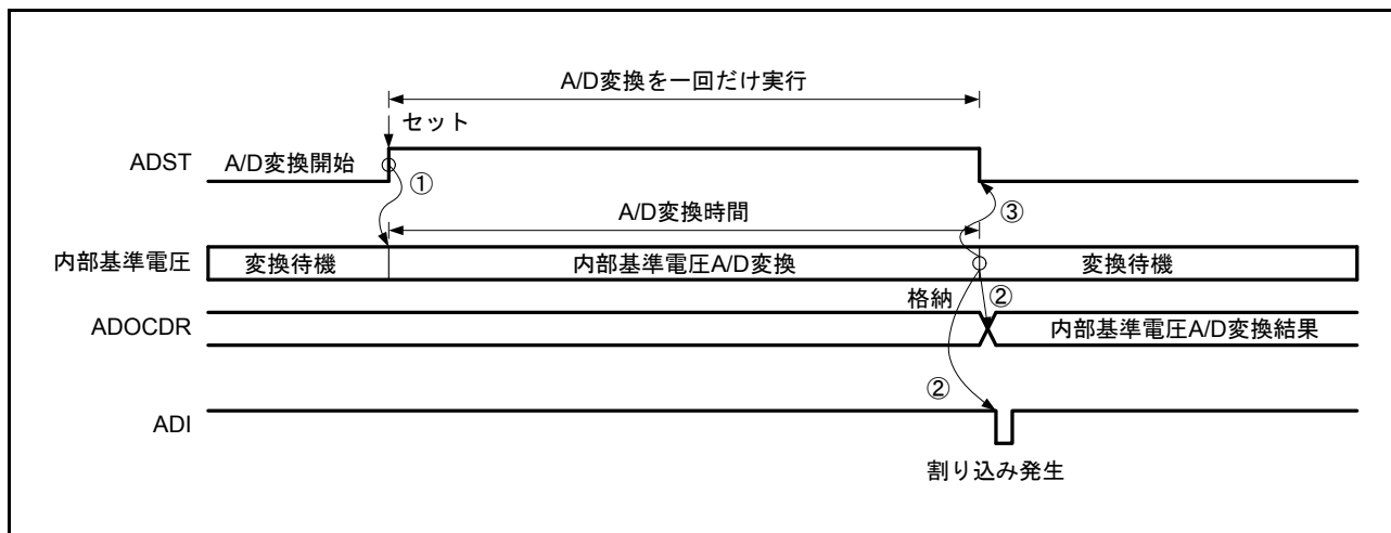
図 35.6 シングルスキャンモードの動作例 (内部基準電圧選択)
