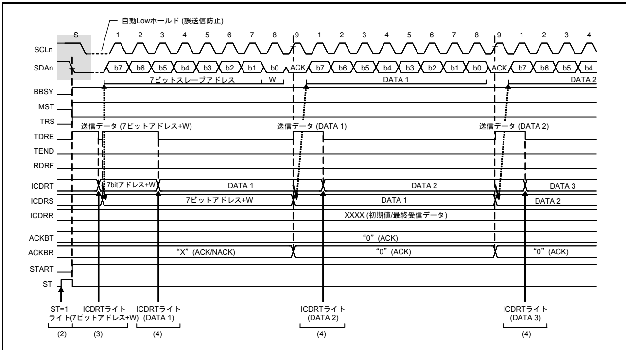
図 31.7 マスタ送信の動作タイミング (1) (7ビットアドレスフォーマットのとき)
