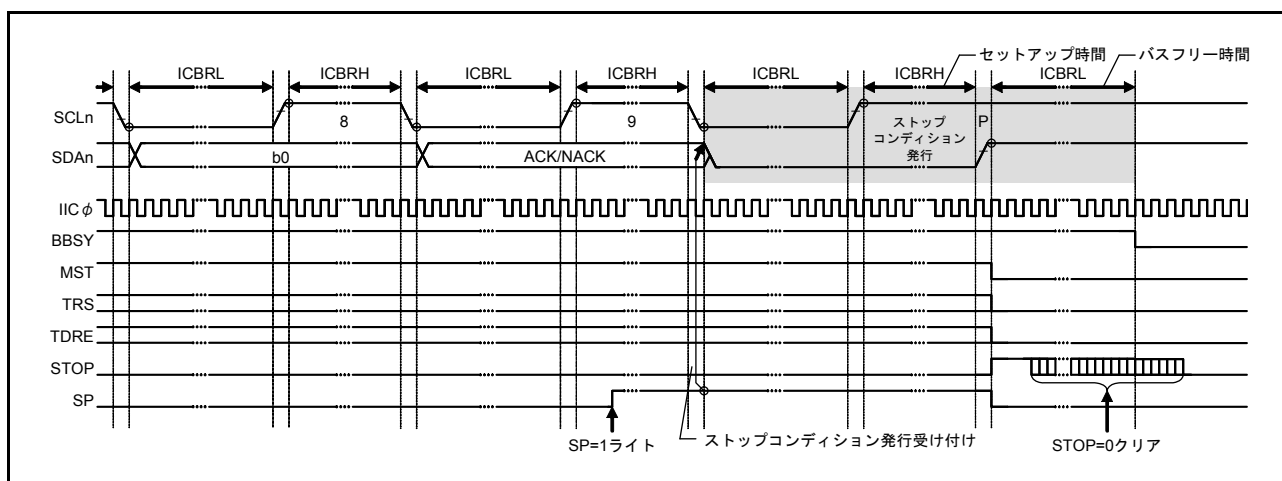
図 31.38 ストップコンディション発行動作タイミング (SPビット)
