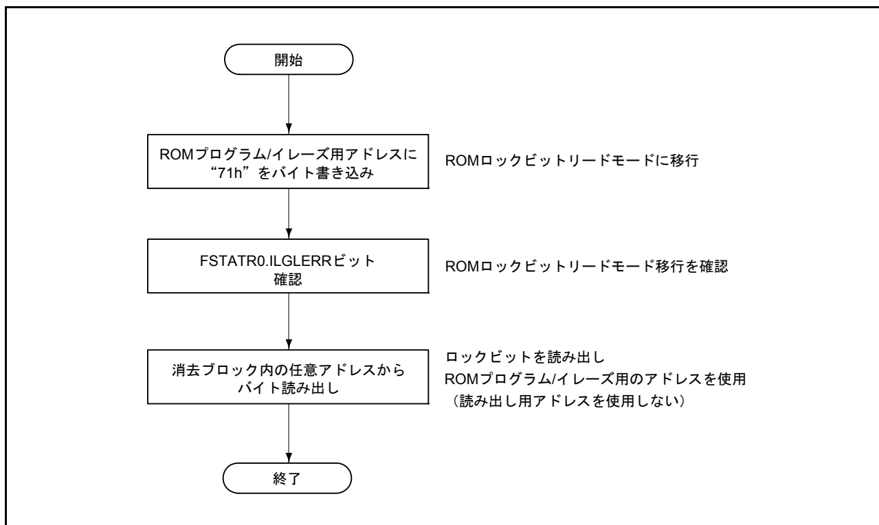
図 42.9 ROM ロックビットリードモード移行フローおよびロックビットを読む方法
