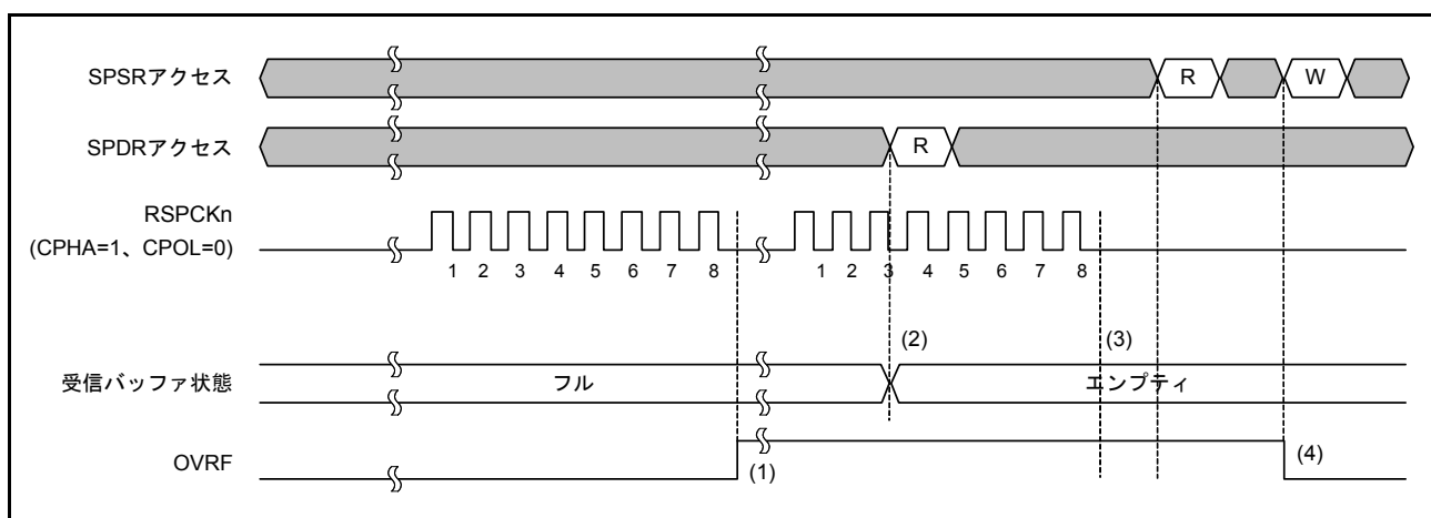
図 32.28 OVRF フラグの動作例
