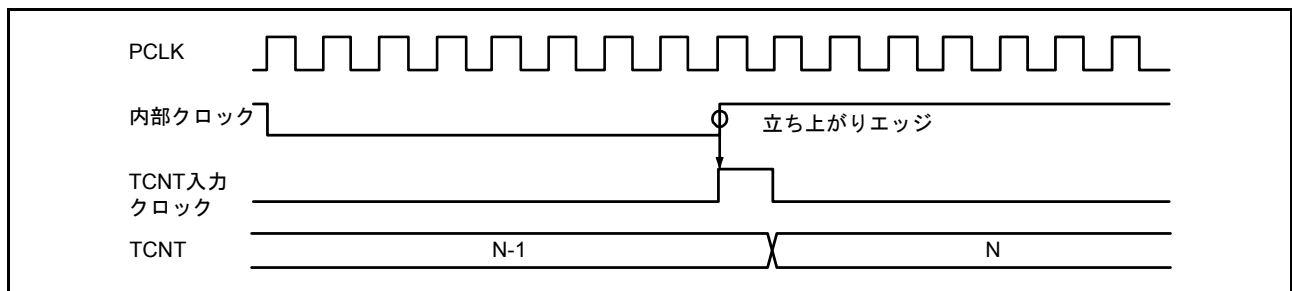
図 22.85 内部クロック動作時のカウントタイミング (MTU5)
