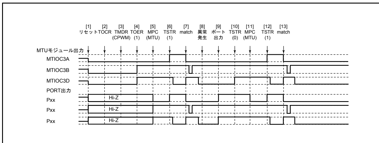
図 22.147 相補 PWM モードで異常が発生し、相補 PWM モードで復帰する場合
