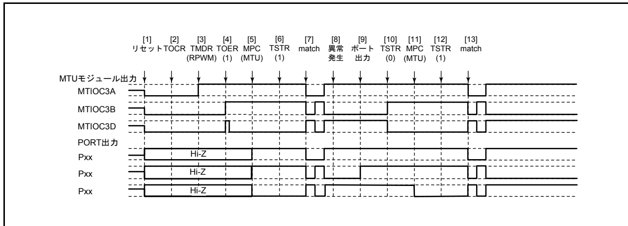
図 22.153 リセット同期 PWM モードで異常が発生し、リセット同期 PWM モードで復帰する場合
