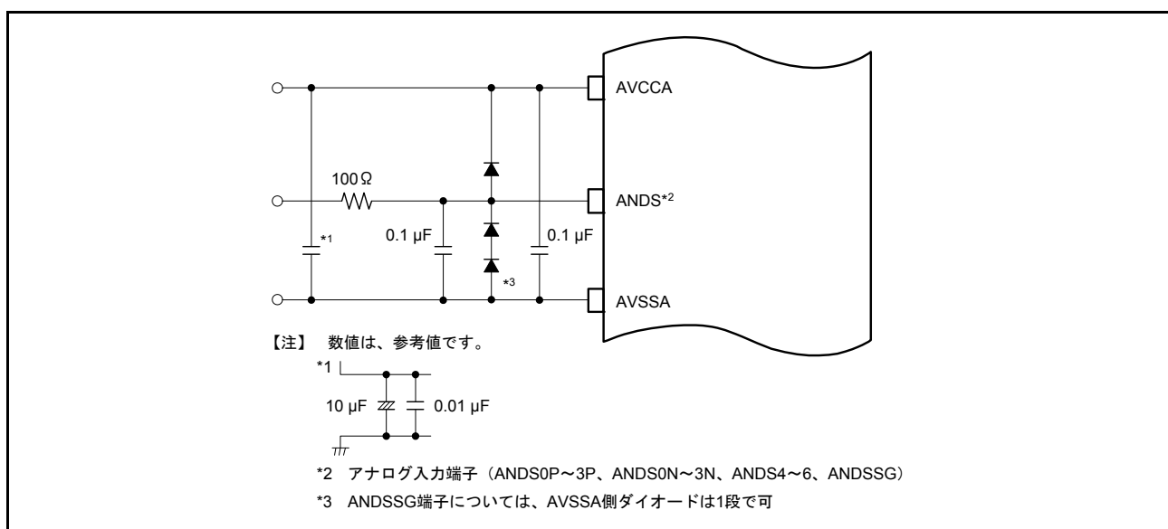
図 34.9 アナログ入力保護回路とアンチエイリアスフィルタの例
