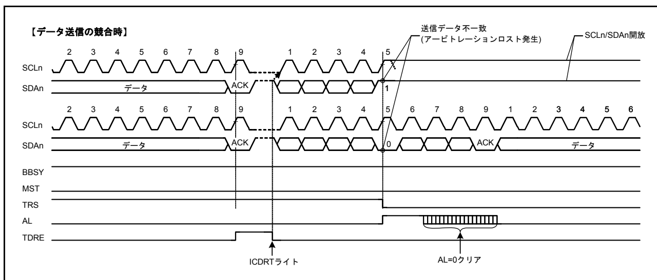
図 31.36 スレーブアービトレーションロスト検出動作例（SALE=1のとき）
