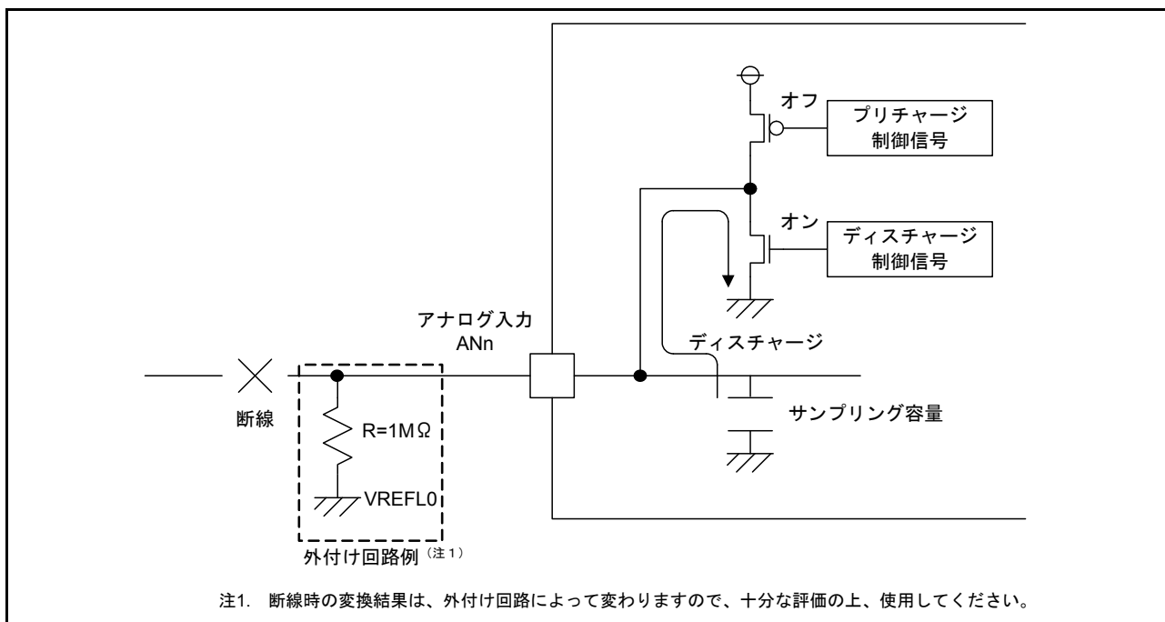
図 35.13 VREFL0 側での断線検出 (ディスチャージを選択)
