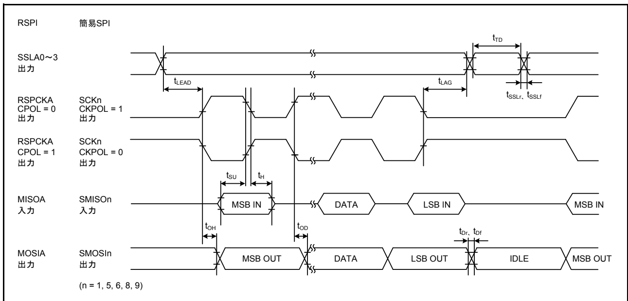
図 44.51 RSPI タイミング (マスタ、CPHA = 1) / 簡易 SPI タイミング (マスタ、CKPH = 0)
