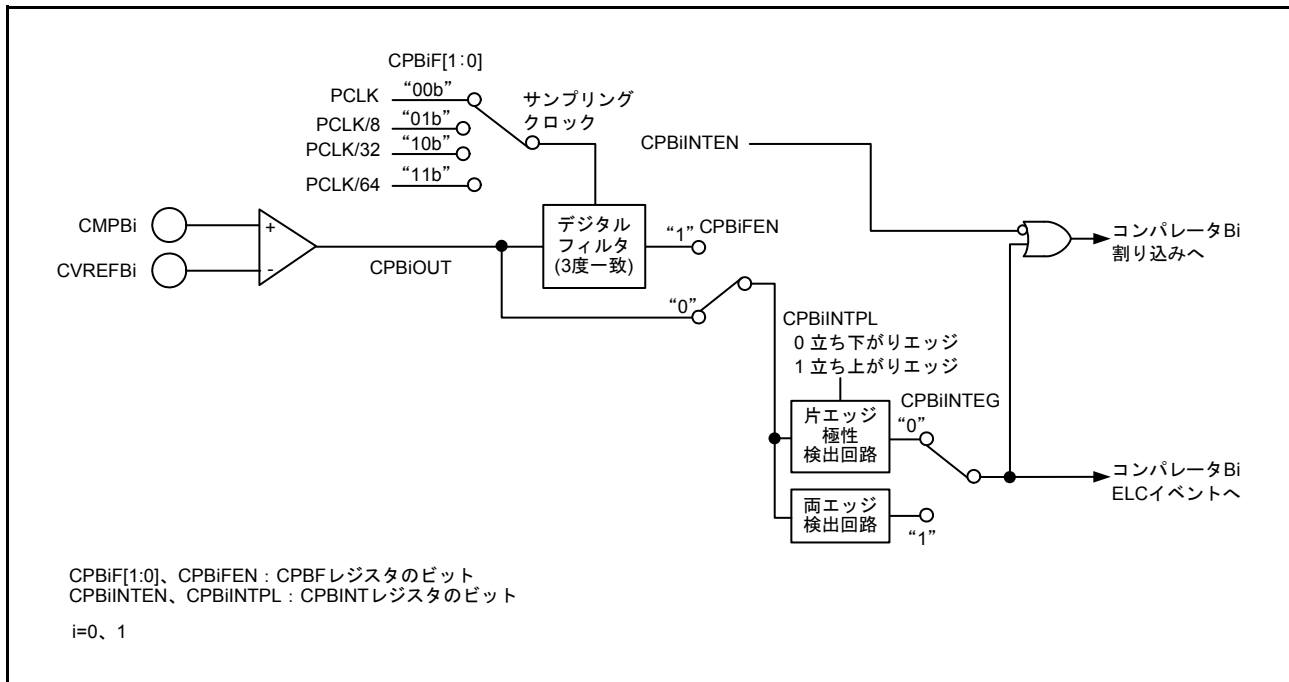
図 39.3 コンパレータ Bi デジタルフィルタの構成
