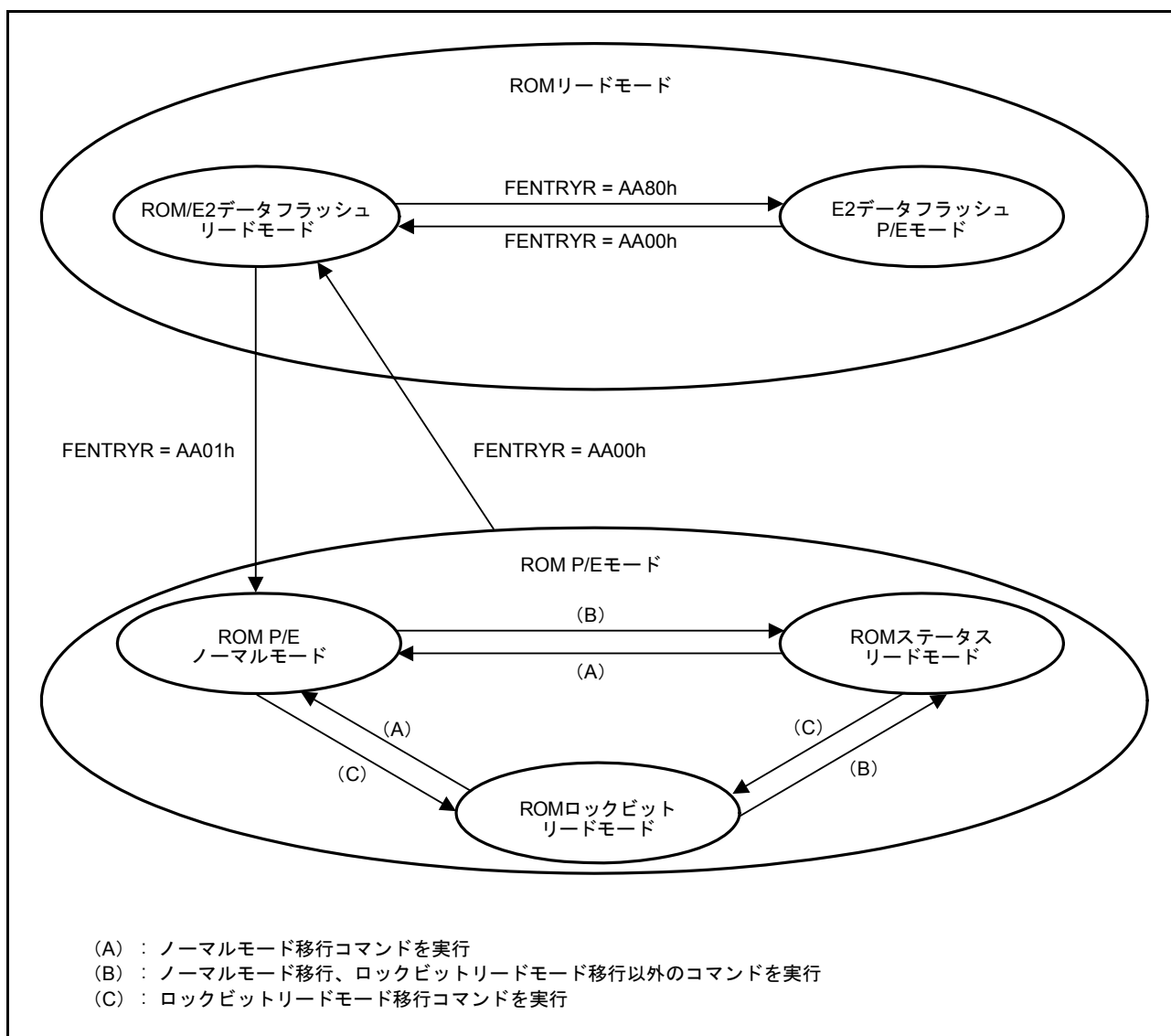
図 42.4 FCU のモード遷移図 (ROM 関連)
