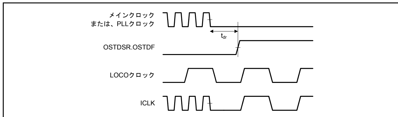
図 44.69 発振停止検出タイミング
