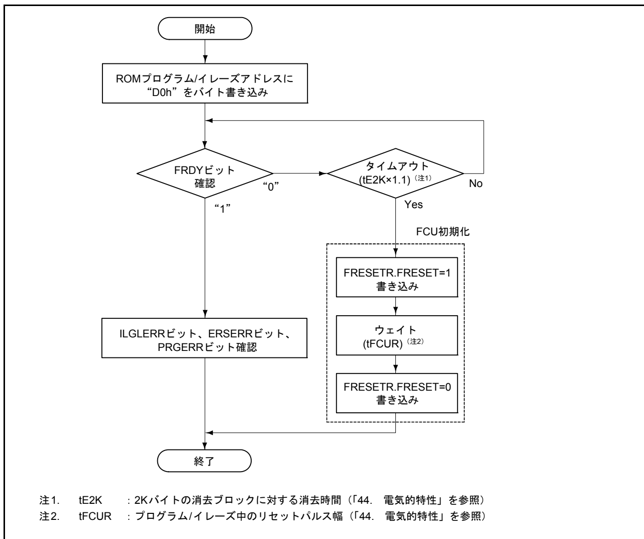
図 42.18 プログラム/イレーズのレジューム方法
