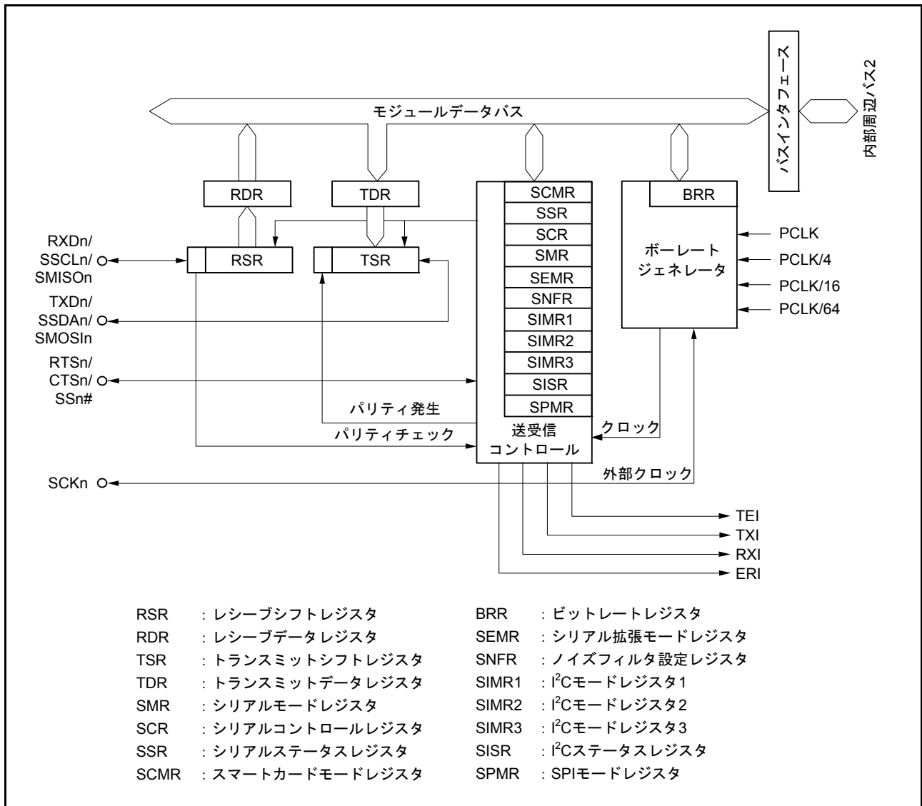
図 29.1 SCI1、8、9 のブロック図
