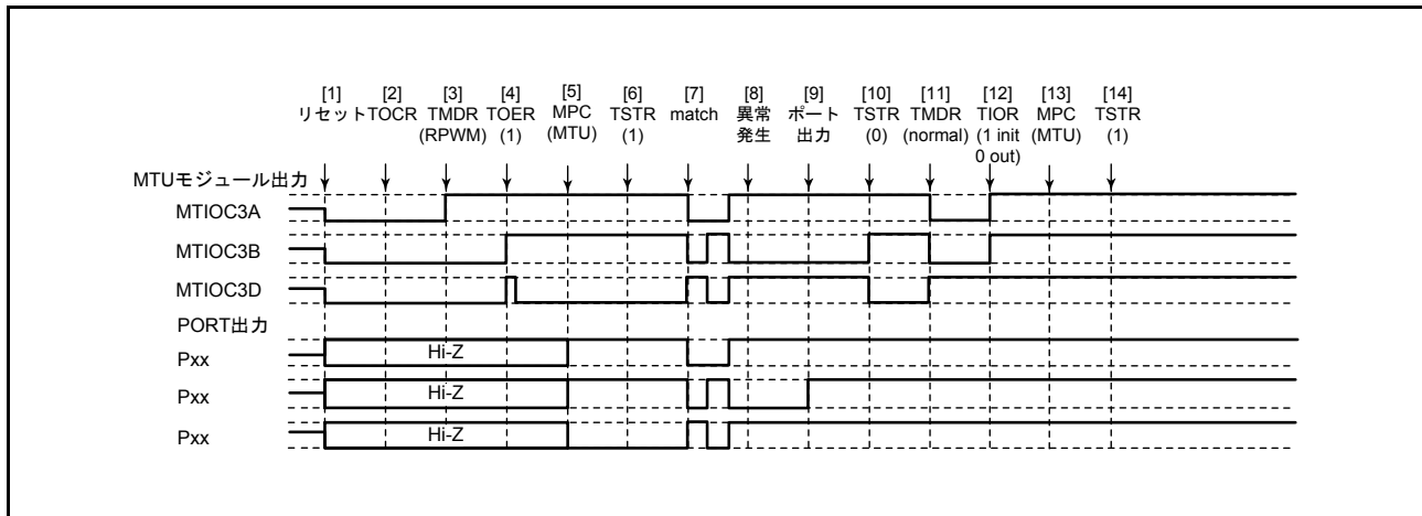
図 22.150 リセット同期 PWM モードで異常が発生し、ノーマルモードで復帰する場合
