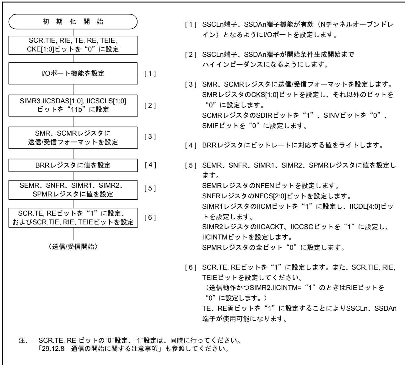
図 29.44 SCIの初期化フローチャート例 (簡易 I 2 C モード)
