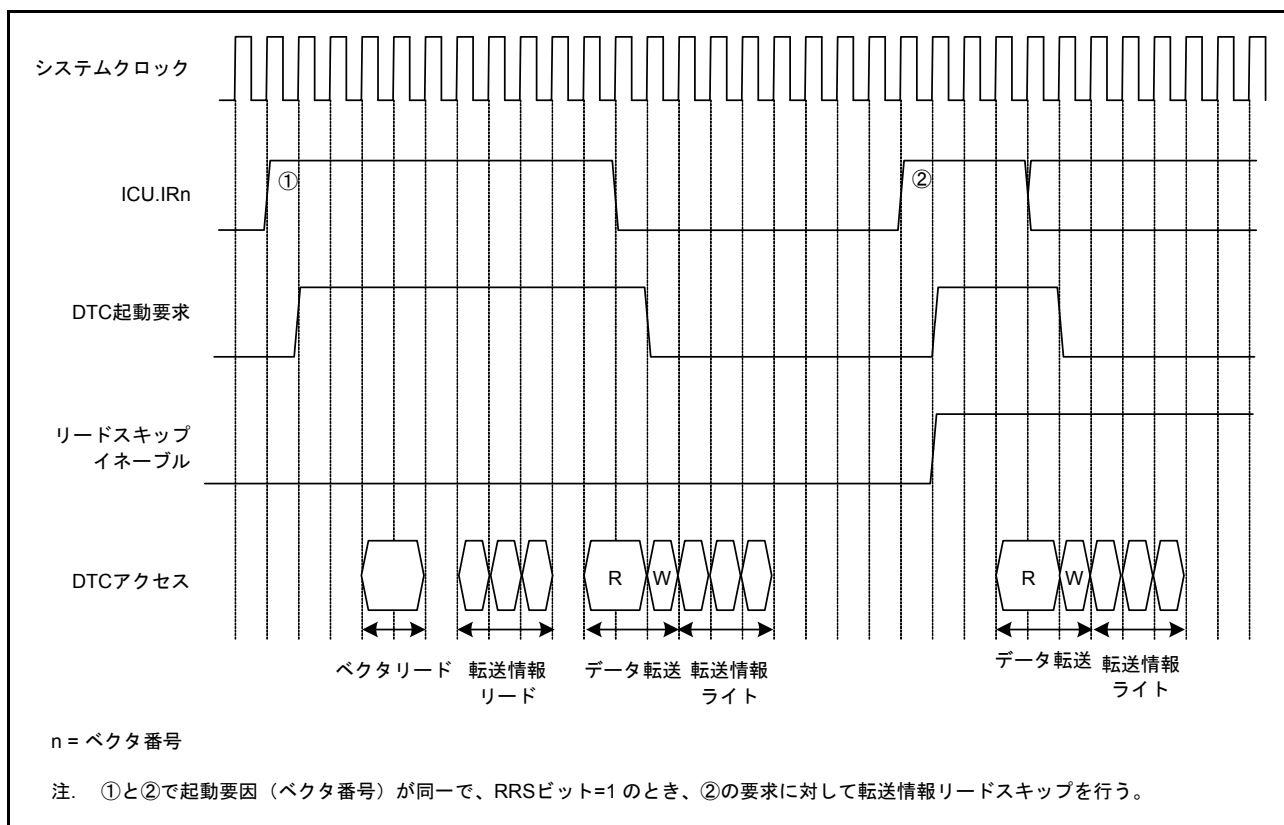
図 18.13 転送情報スキップ時の動作例 (ベクタ、転送情報、転送先が RAM、転送元は周辺モジュールの場合)
