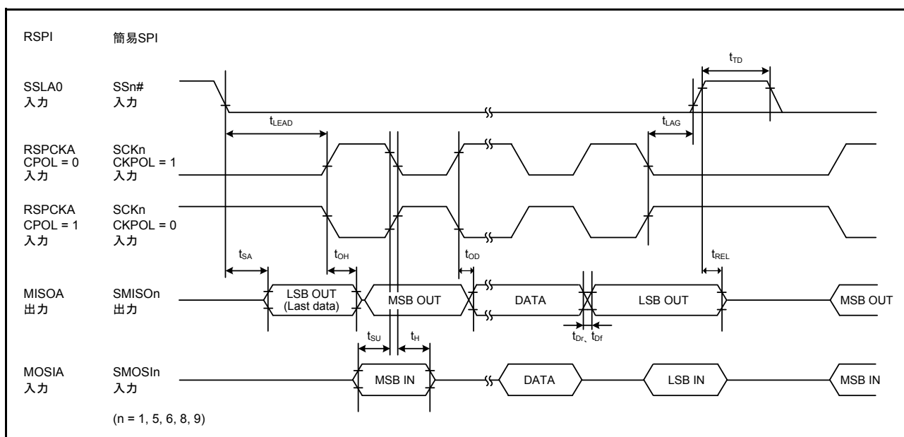
図 44.53 RSPI タイミング (スレーブ、CPHA = 1) / 簡易 SPI タイミング (スレーブ、CKPH = 0)
