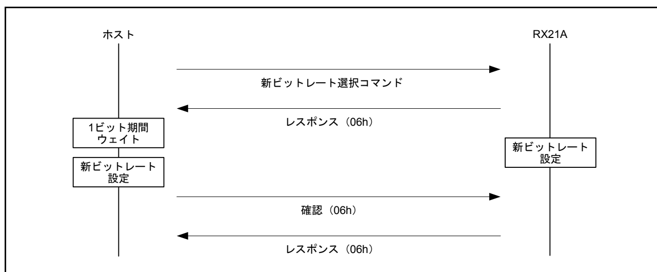
図 42.27 新ビットレート選択のシーケンス
