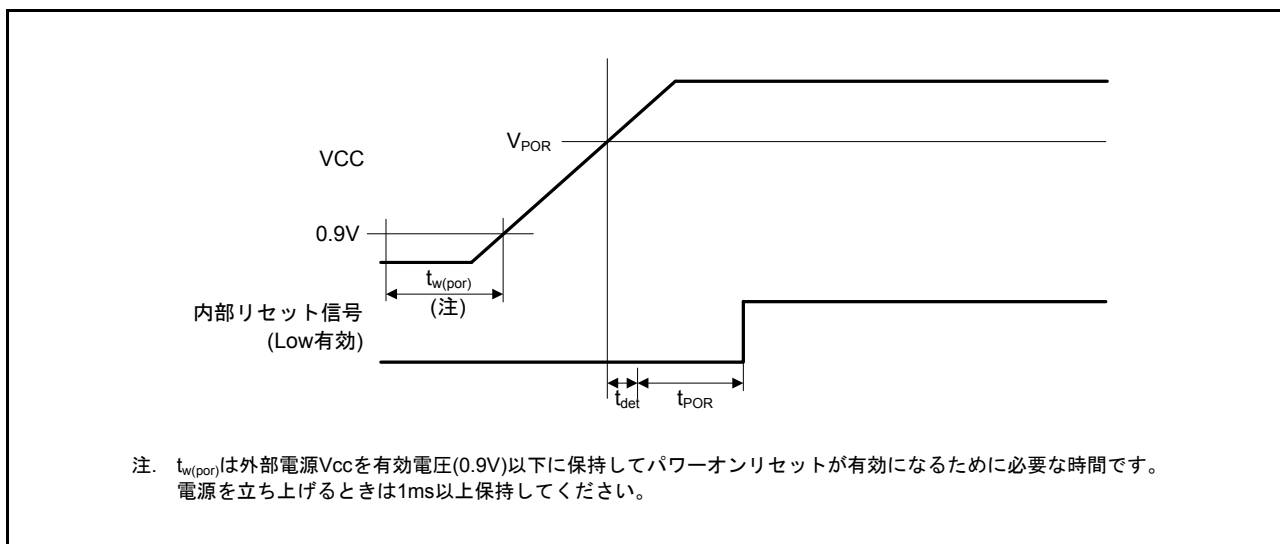
図 44.65 パワーオンリセットタイミング
