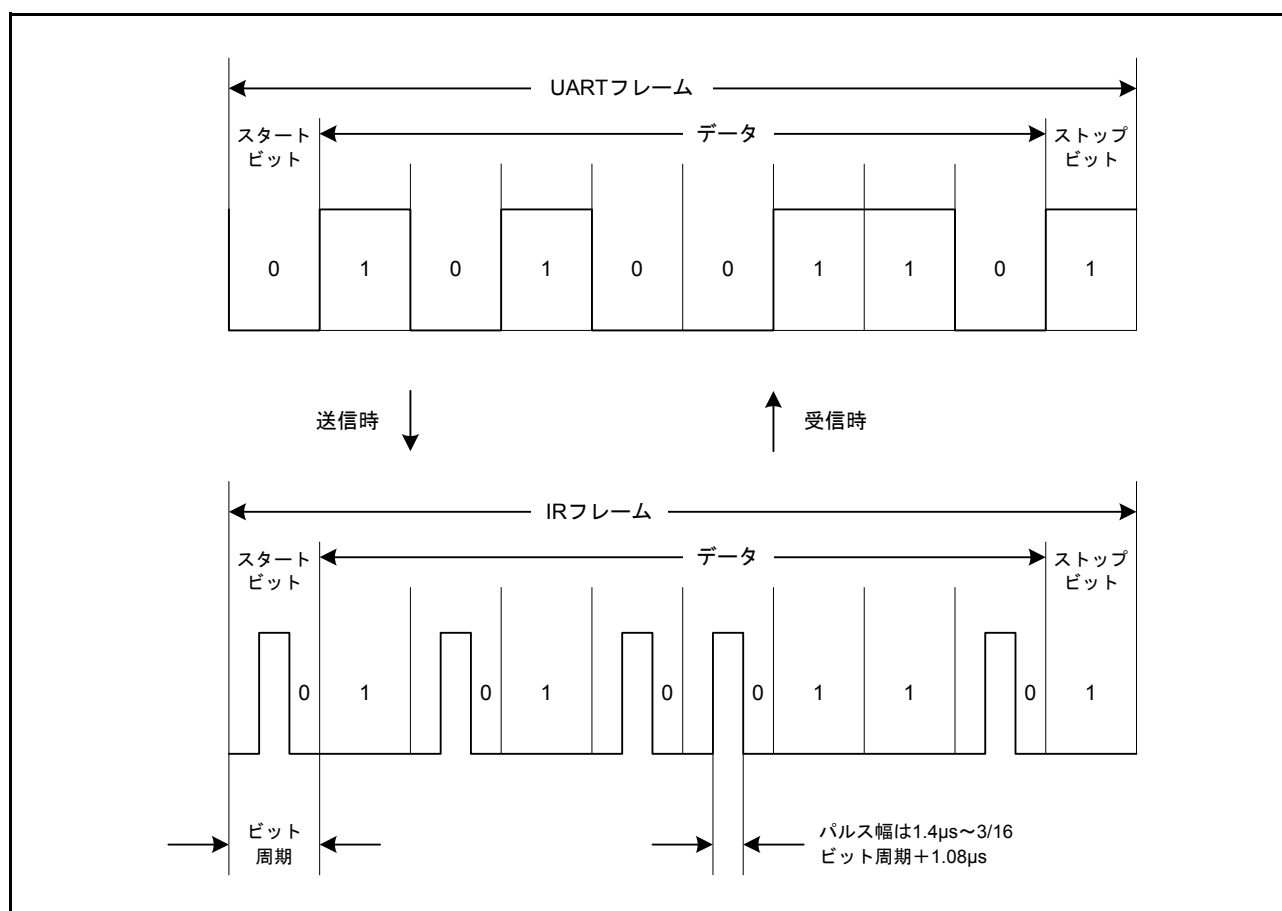
図 30.2 IrDA の送信 / 受信動作図
