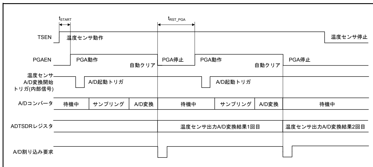
図 44.63 温度センサの A/D 変換タイミング例 (2 変換の場合)
