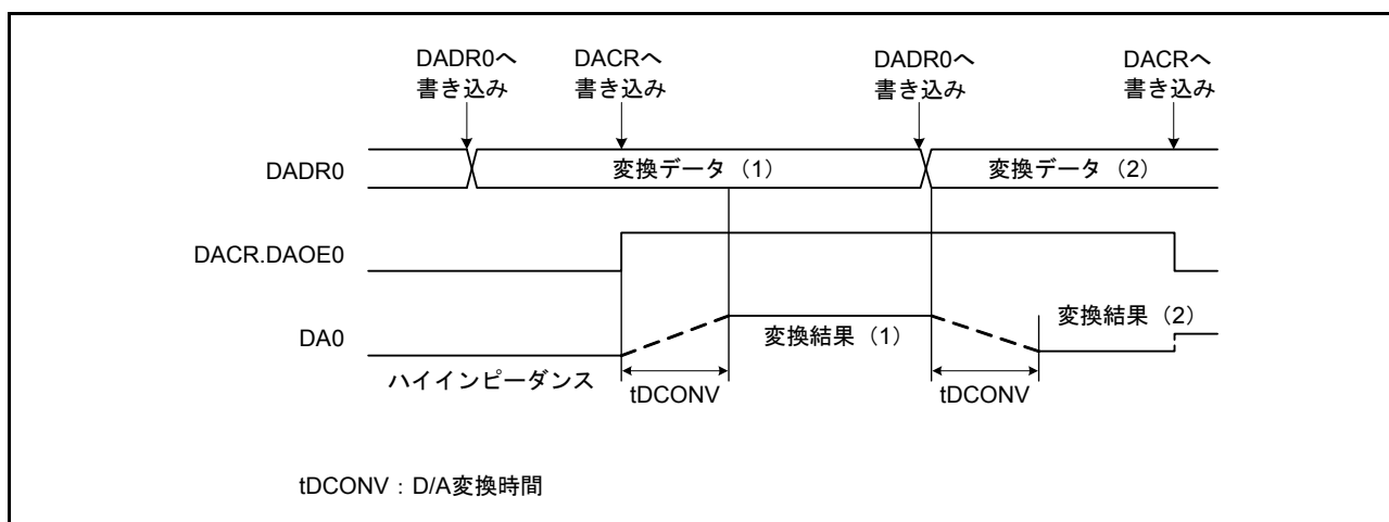
図 36.2 D/Aコンバータの動作例
