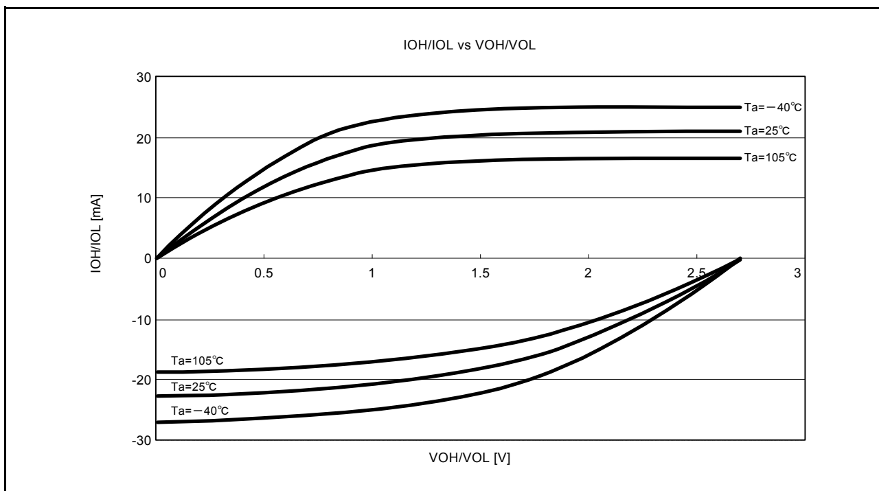
図 44.18 高駆動出力を選択したときの VOH/VOL IOH/IOL 温度特性 VCC = 2.7V (参考データ)
