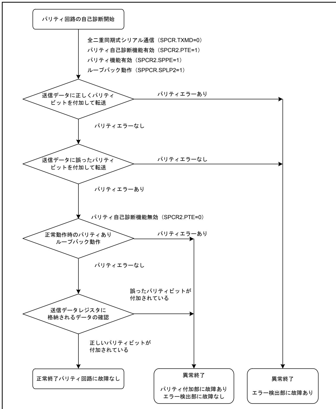
図 32.48 パリティ回路の自己判断フロー
