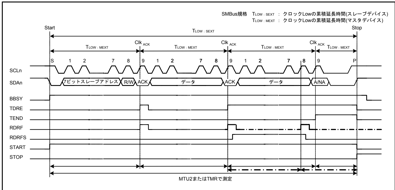
図 31.41 SMBus タイムアウト測定
