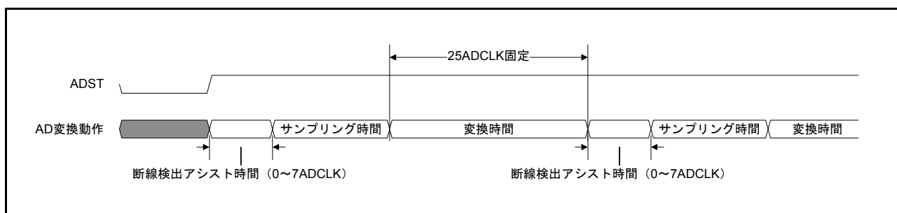
図 35.11 断線検出アシスト機能を使用した場合の A/D 変換動作図
