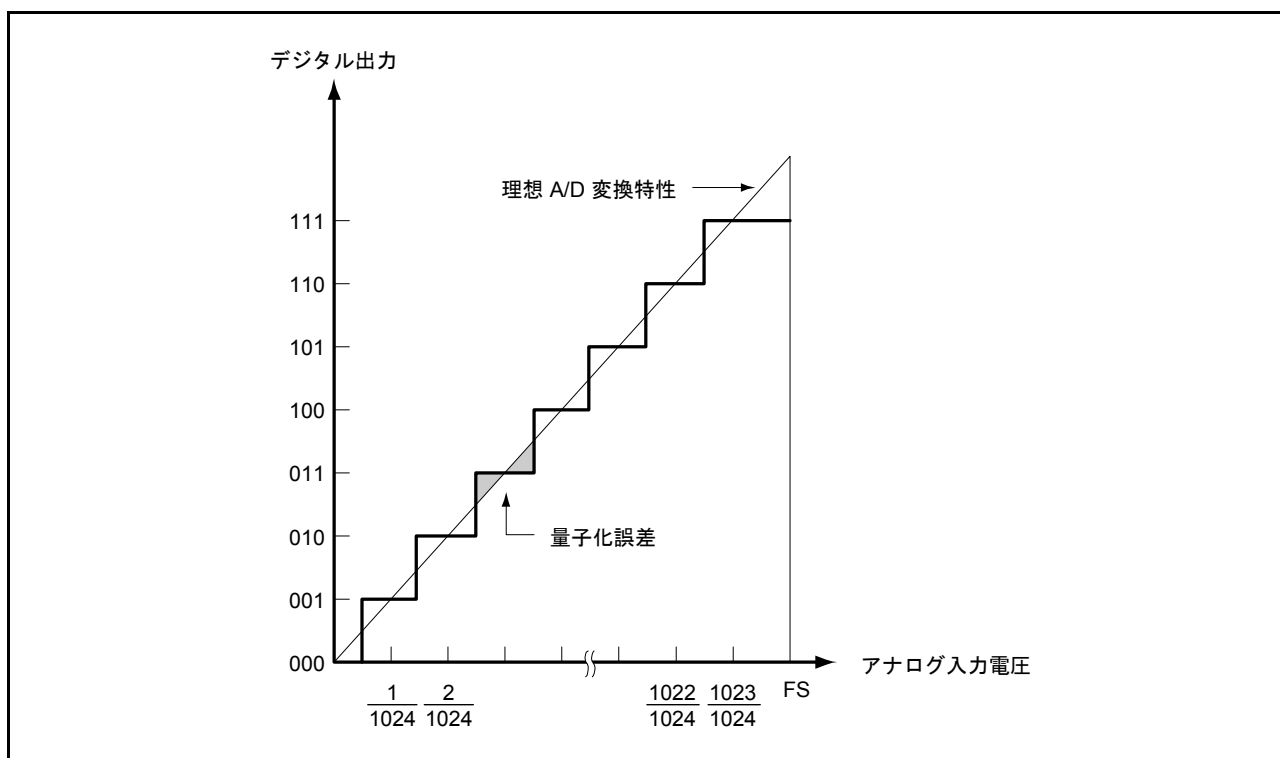
図 35.15 A/D 変換精度の定義 (1)
