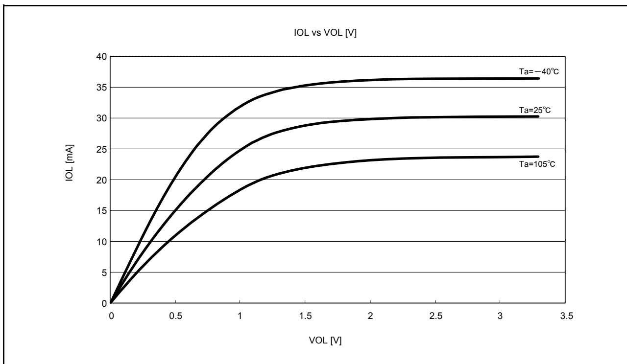
図 44.23 RIIC 出力端子の VOL、IOL 温度特性 VCC=3.3V (参考データ)
