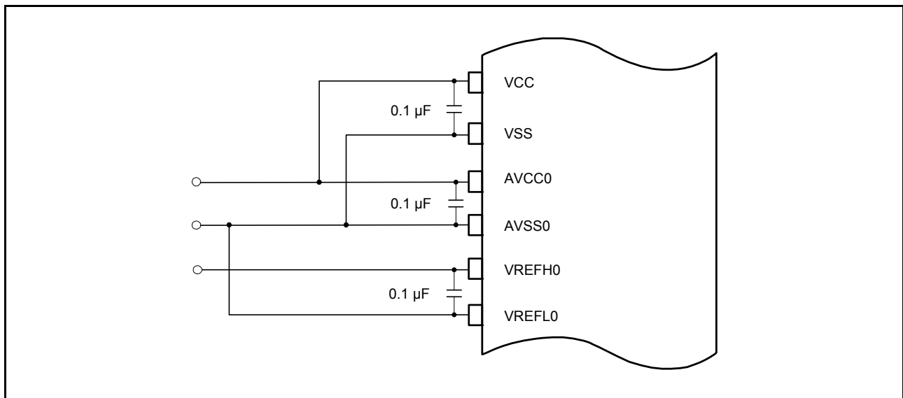
図 35.18 各電源端子の接続例
