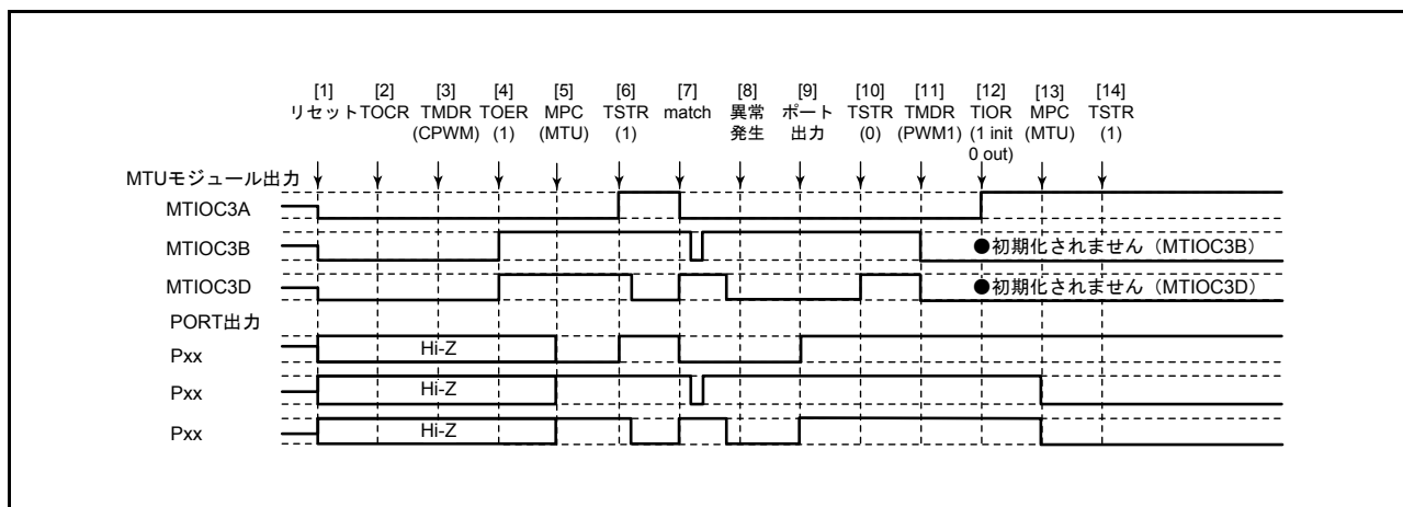
図 22.146 相補 PWM モードで異常が発生し、PWM モード 1 で復帰する場合
