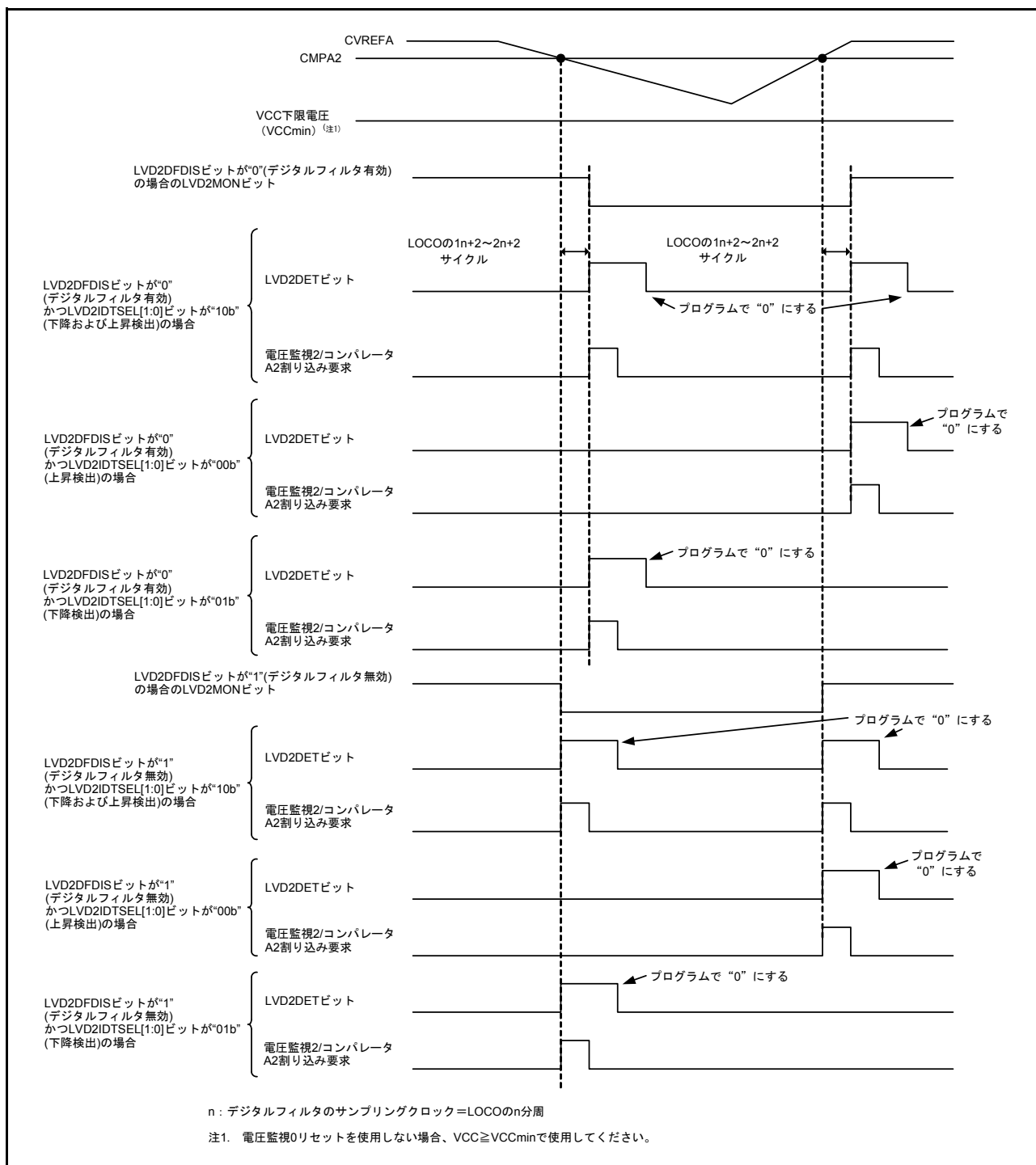
図 38.3 コンパレータ A2 動作例
