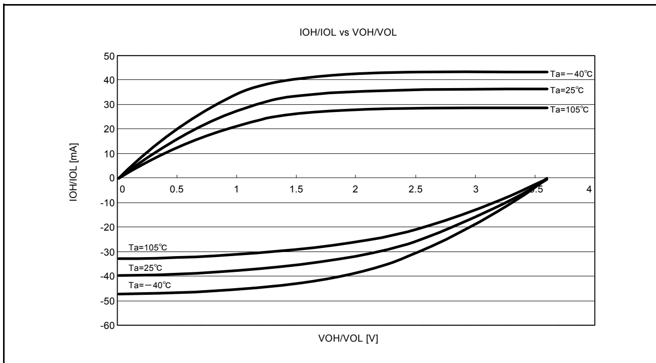
図 44.20 高駆動出力を選択したときの VOH/VOL IOH/IOL 温度特性 VCC = 3.6V (参考データ)
