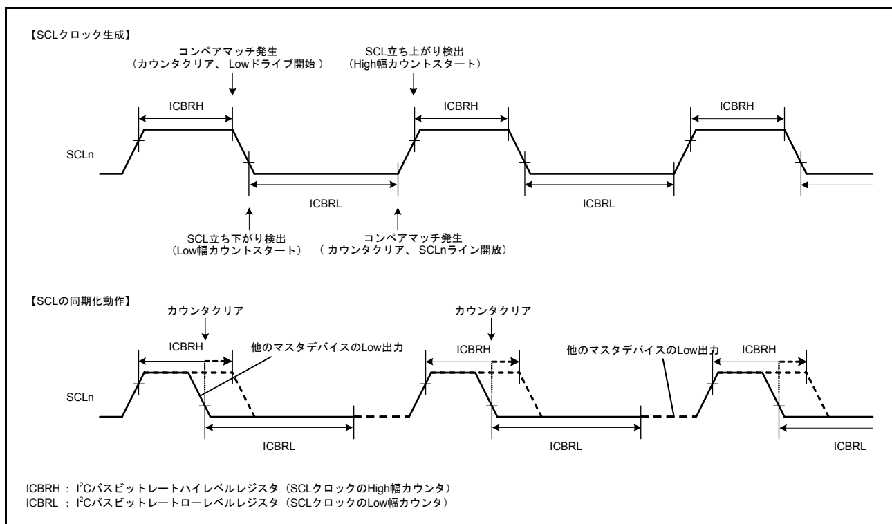
図 31.21 RIIC の SCL クロック生成および SCL 同期化動作
