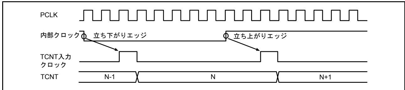
図 22.84 内部クロック動作時のカウントタイミング (MTU0 ~ MTU4)
