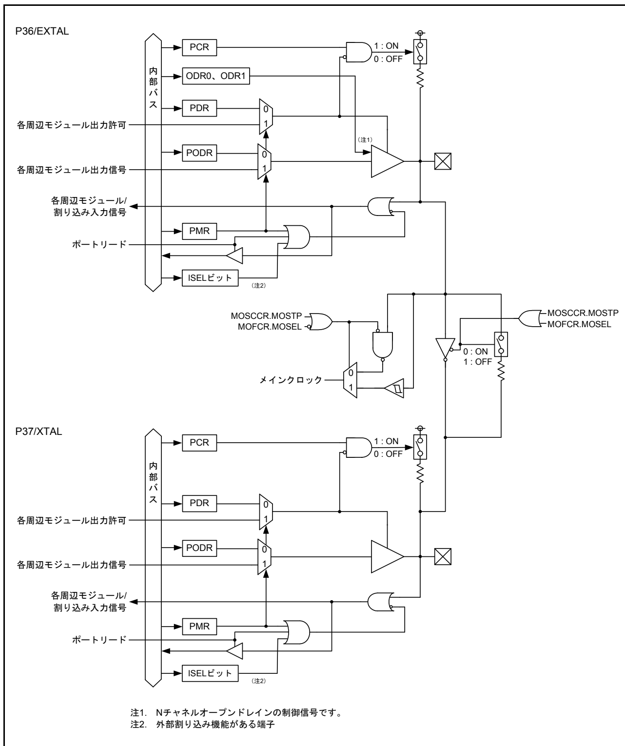
図 20.6 入出力ポートの構成 (6)
