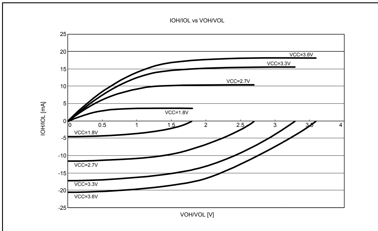
図 44.11 通常出力を選択したときの VOH/VOL、IOH/IOL 電圧特性 T_a = 25^\circ\text{C} (参考データ)
