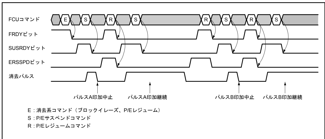
図 42.19 消去処理の中断動作（サスペンド優先モード）
