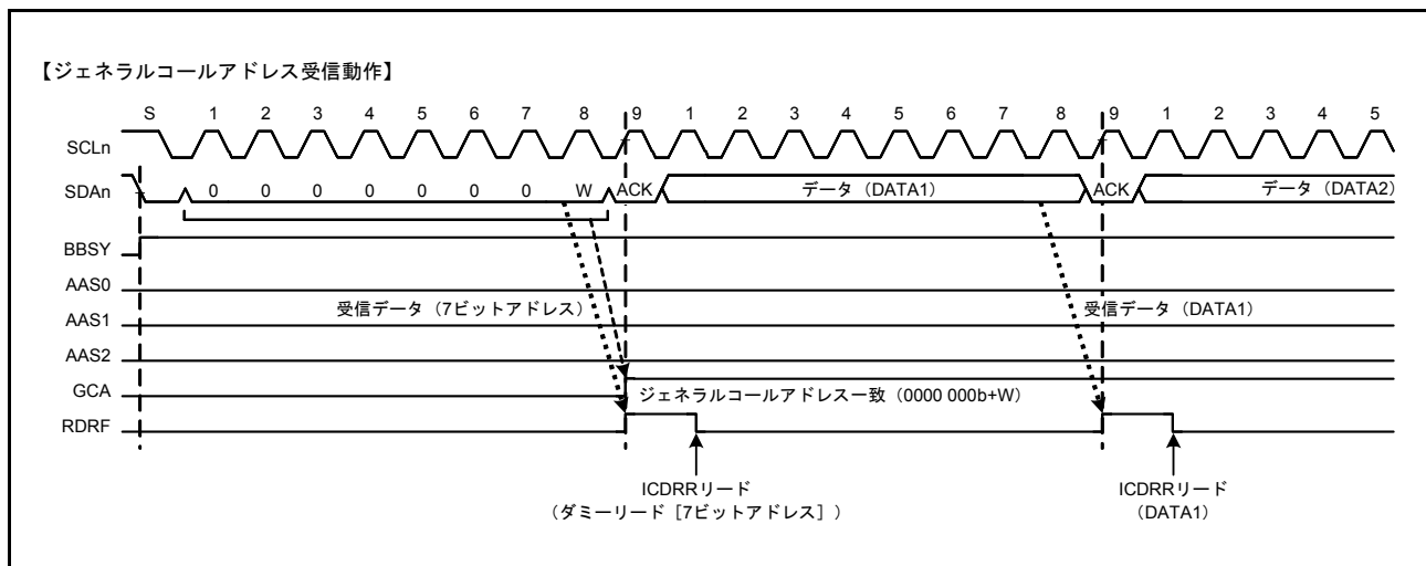
図 31.27 ジェネラルコールアドレス受信時に GCA フラグが“1”になるタイミング
