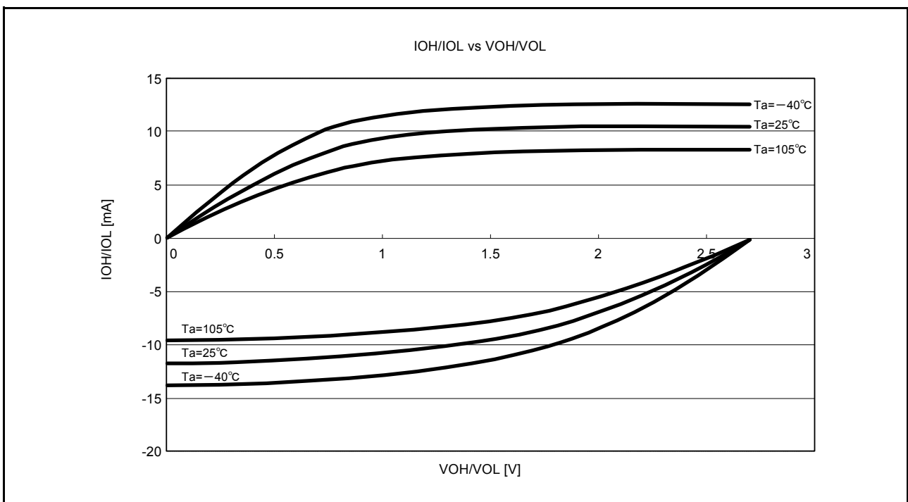
図 44.13 通常出力を選択したときの VOH/VOL IOH/IOL 温度特性 VCC = 2.7V (参考データ)
