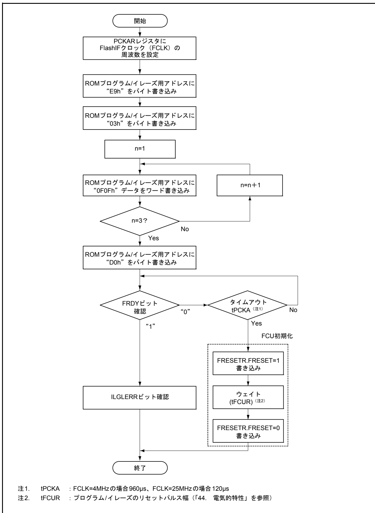
図 42.11 周辺クロック通知コマンドの使用法
