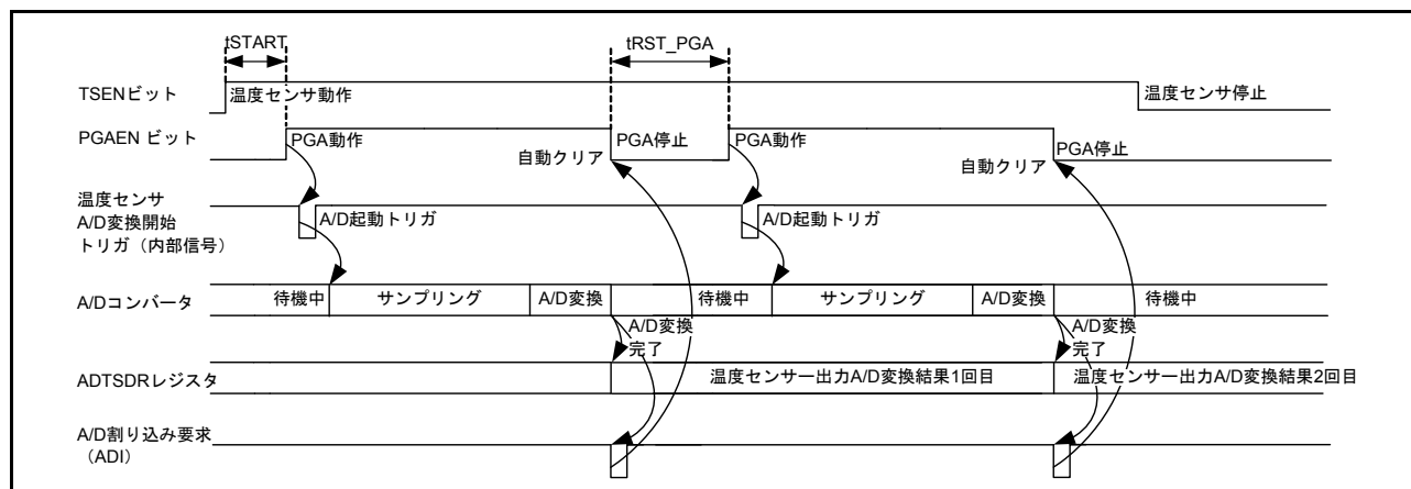
図 37.4 温度センサの A/D 変換タイミング例 (2 変換の場合)
