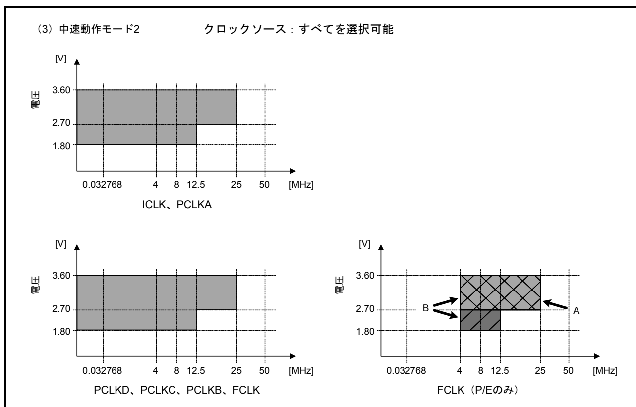
図 11.4 中速動作モード 2A、2B における動作電圧と動作周波数の関係
