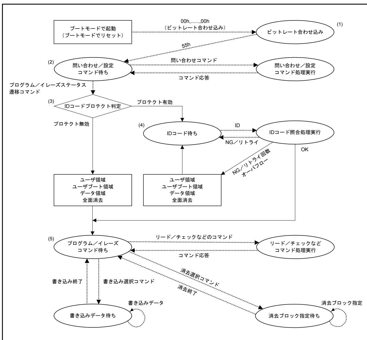
図 42.22 ブートモードの状態遷移図
