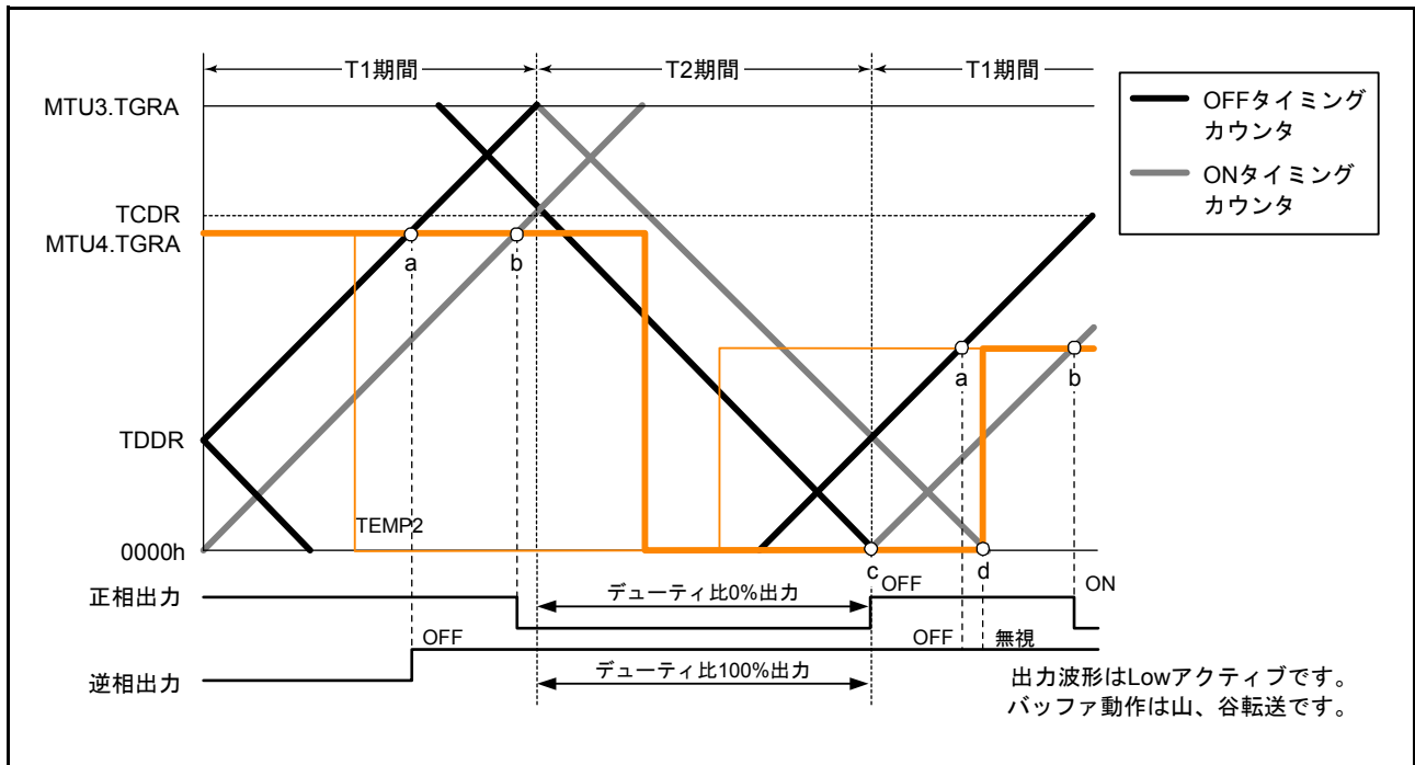
図 22.51 相補 PWM モード 0%、100% 波形出力例 (3)
