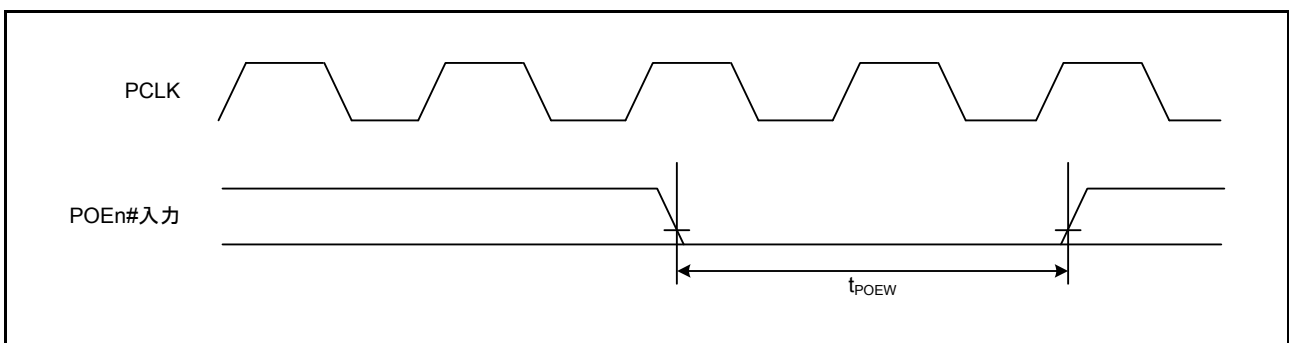
図 44.44 POE# 入力タイミング
