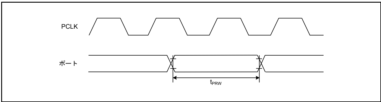
図 44.41 I/O ポート入力タイミング
