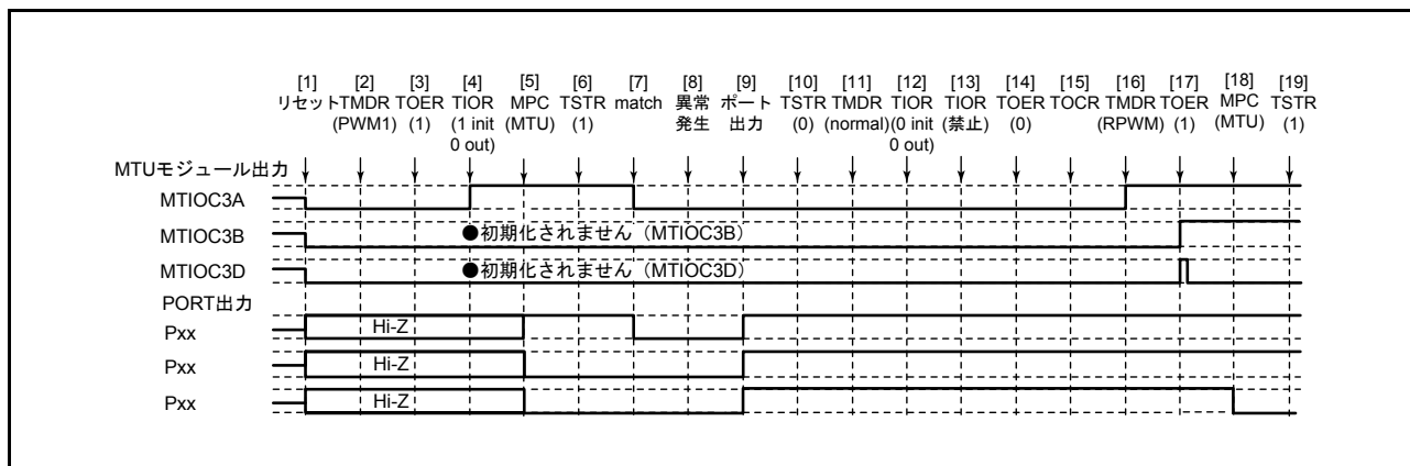
図 22.136 PWM モード 1 で異常が発生し、リセット同期 PWM モードで復帰する場合
