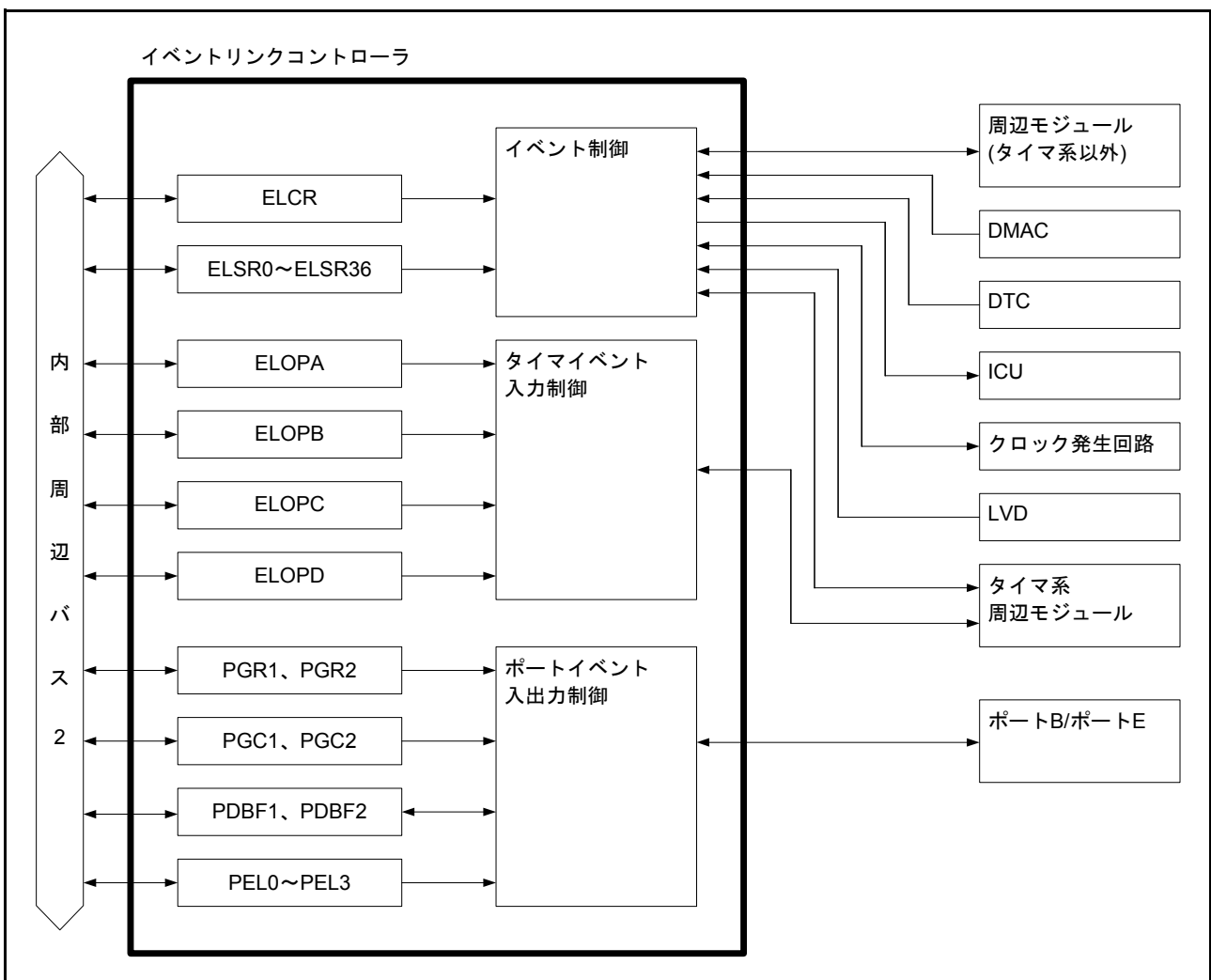
図 19.1 ELCのブロック図
