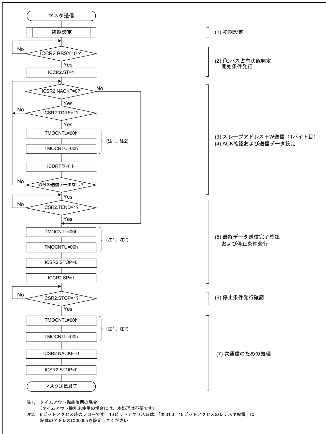
図 31.6 マスタ送信のフローチャート例
