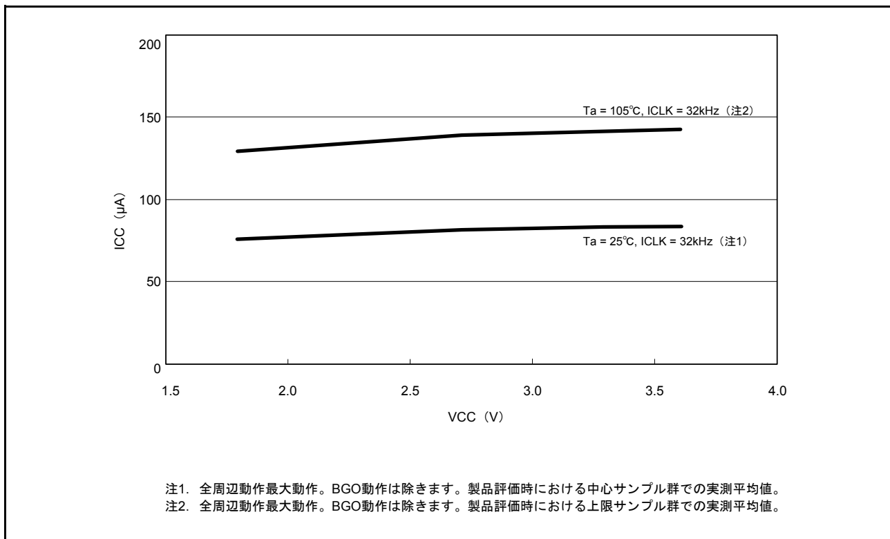
図 44.5 低速動作モード2の電圧依存性（参考データ）
