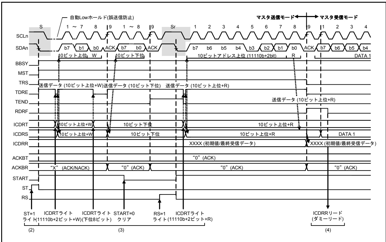
図 31.13 マスタ受信の動作タイミング (2) (10ビットアドレスフォーマット、RDRFS=0 のとき)
