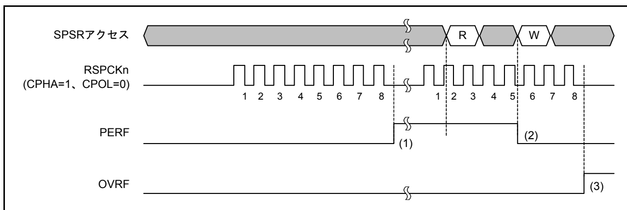
図 32.29 PERF フラグの動作例
