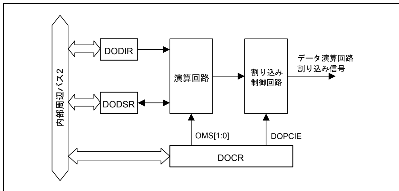
図 40.1 データ演算回路のブロック図
