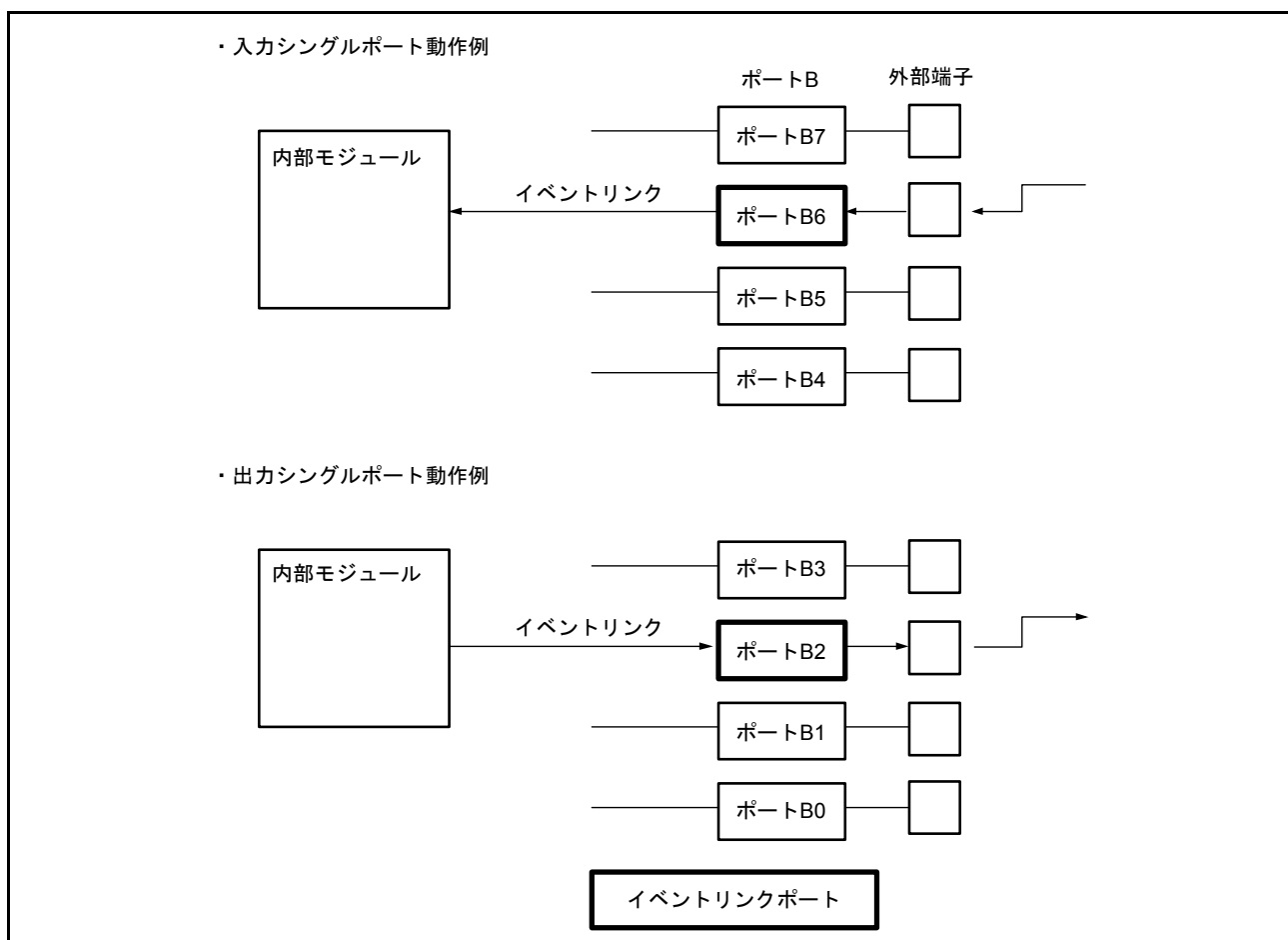
図 19.3 シングルポートのイベントリンク動作
