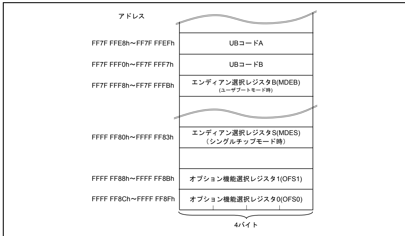
図 7.1 オプション設定メモリ領域
