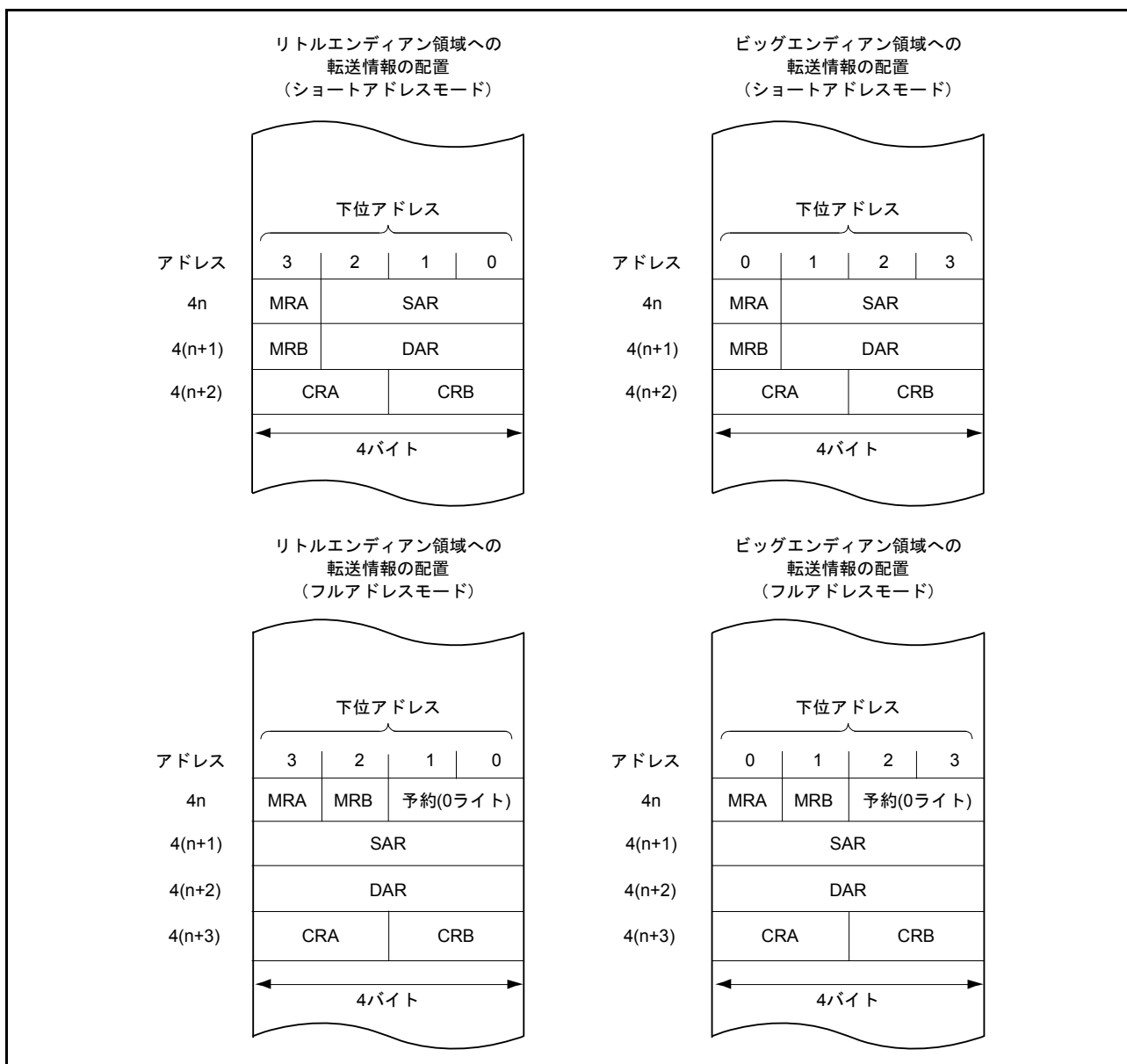
図 18.16 転送情報の配置
