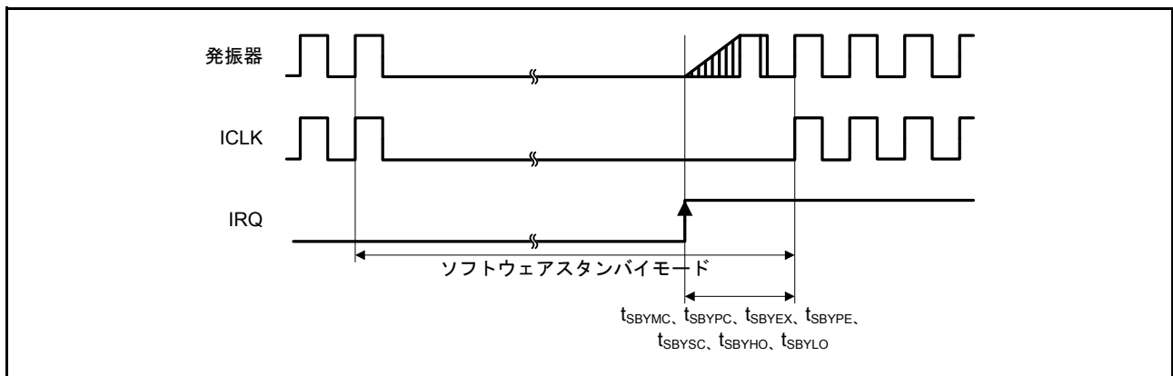
図 44.37 ソフトウェアスタンバイモード解除タイミング
