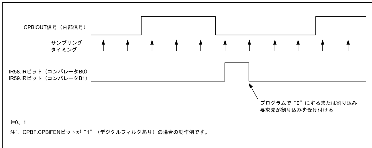
図 39.4 コンパレータ Bi デジタルフィルタ動作例
