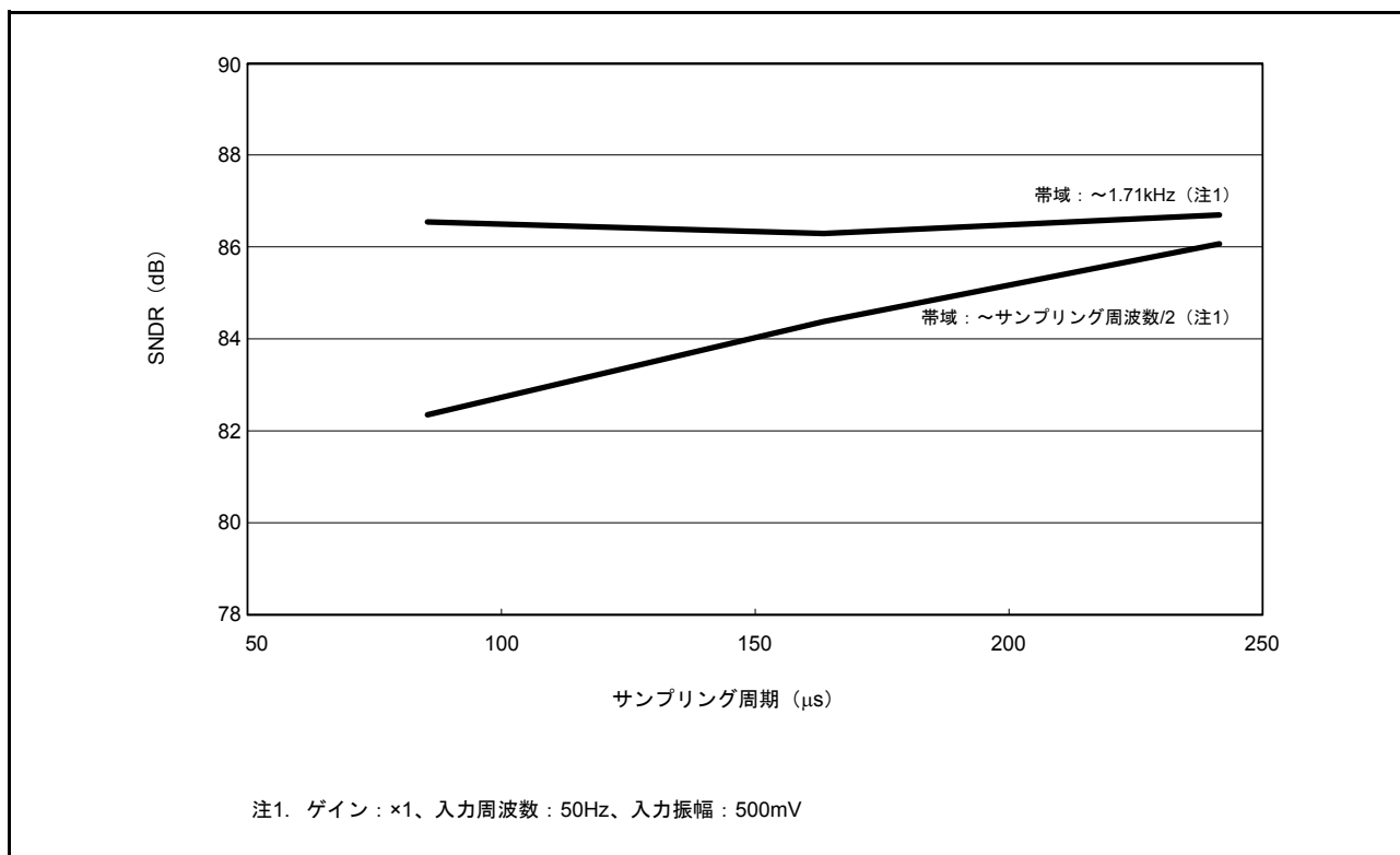
図 44.58 SNDR のサンプリング周期依存性 (参考データ)
