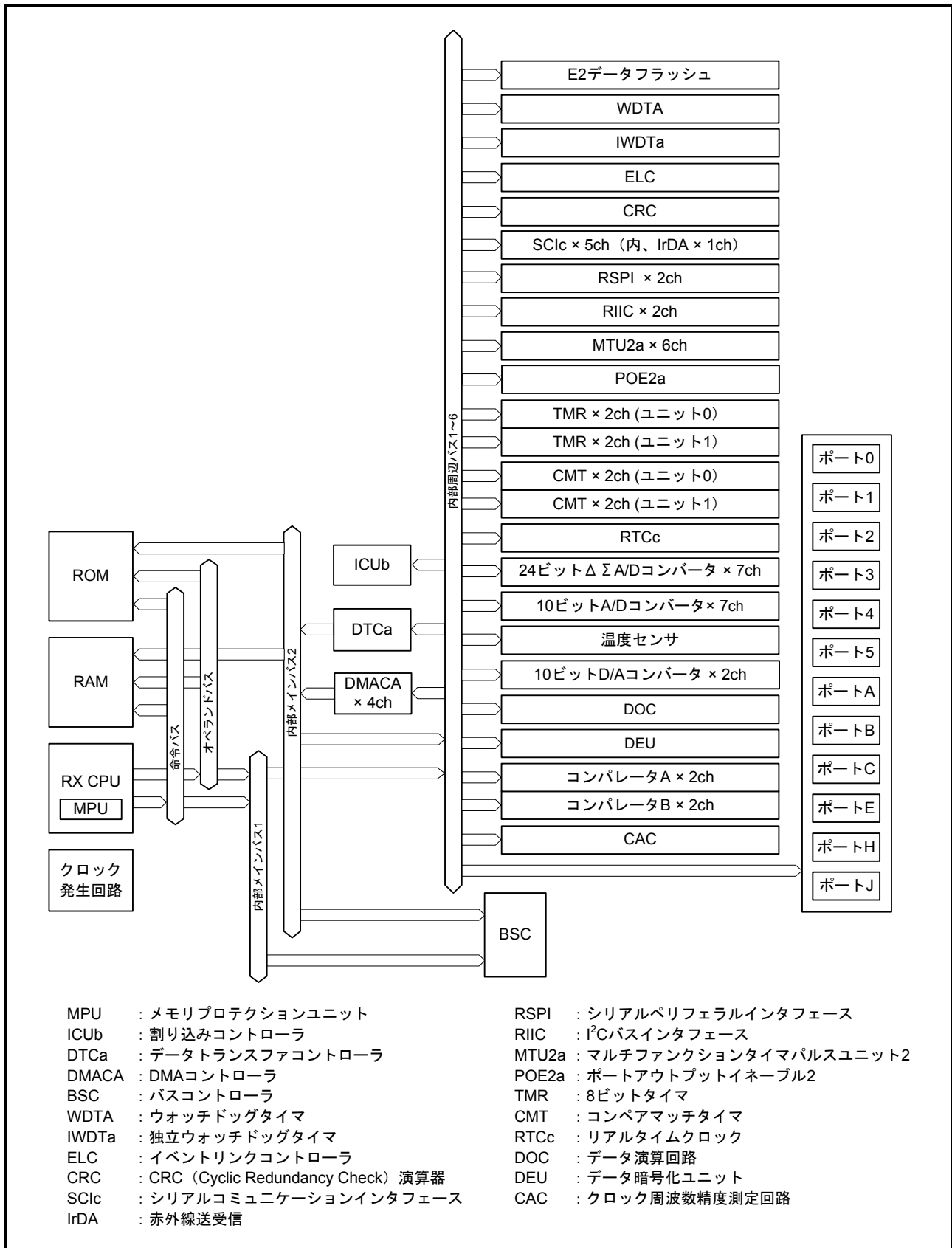
図 1.2 100 ピン版のブロック図
