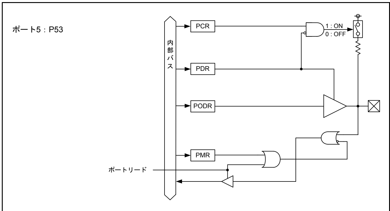
図 20.5 入出力ポートの構成 (5)
