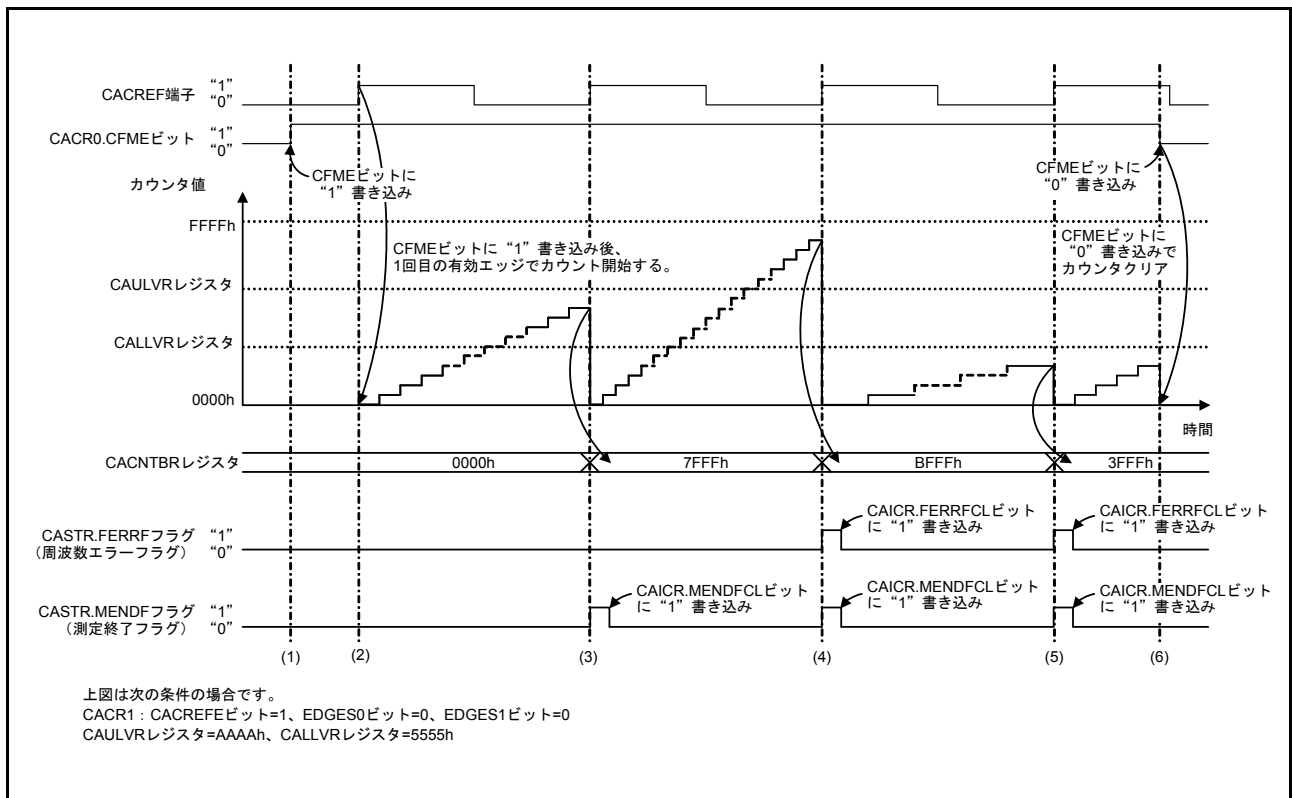
図 10.2 CACREF 端子入力を基準としたクロック周波数精度測定回路の動作例
