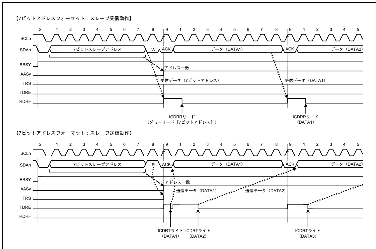
図31.24 7ビットアドレスフォーマット選択時にAASyフラグが“1”になるタイミング
