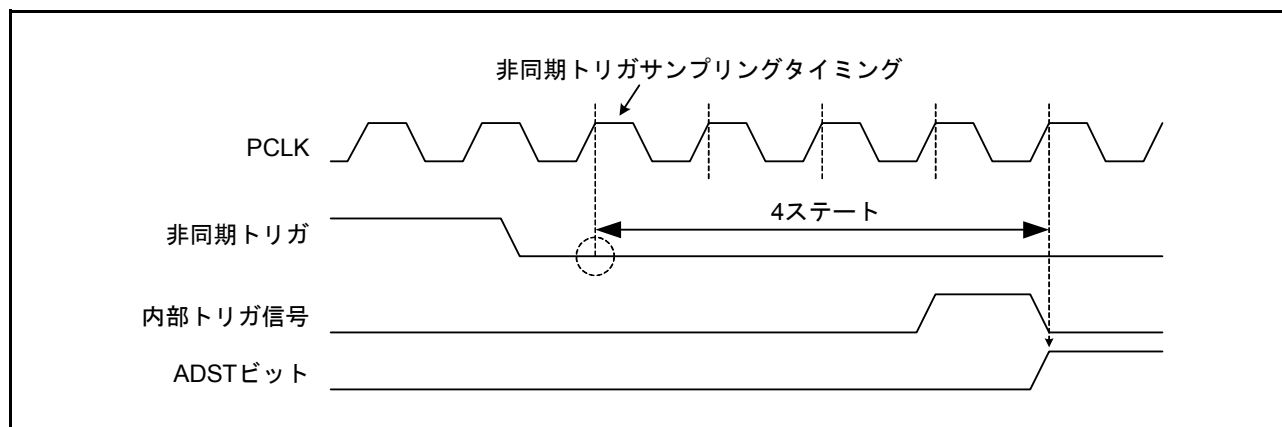
図 35.14 非同期トリガ入力タイミング
