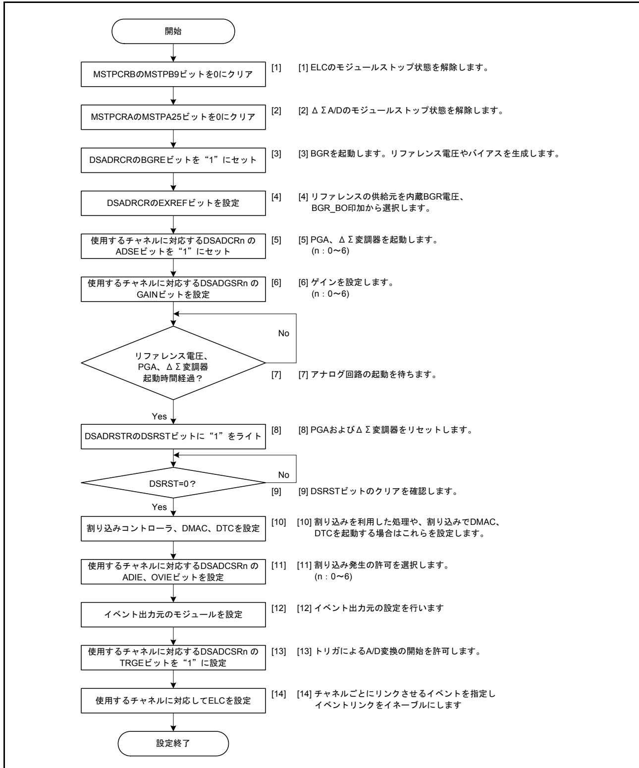
図 34.2 \Delta\Sigma A/Dコンバータの起動手順
