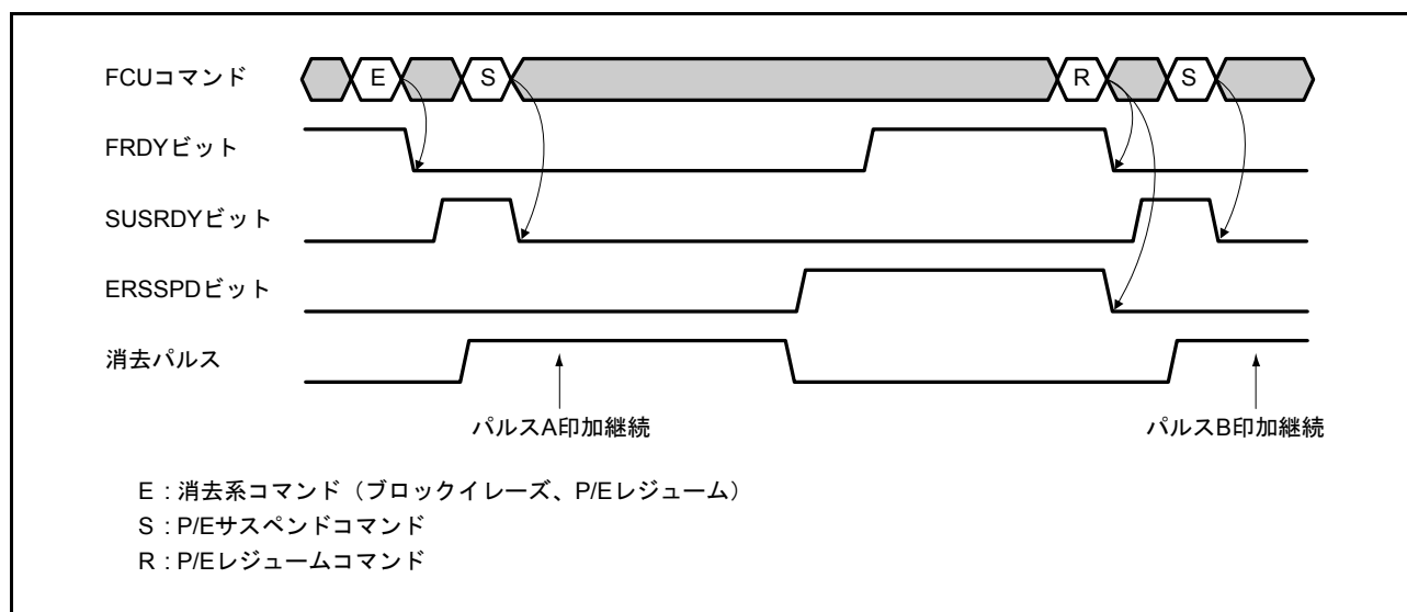
図 42.20 消去処理の中断動作（書き込み / 消去優先モード）
