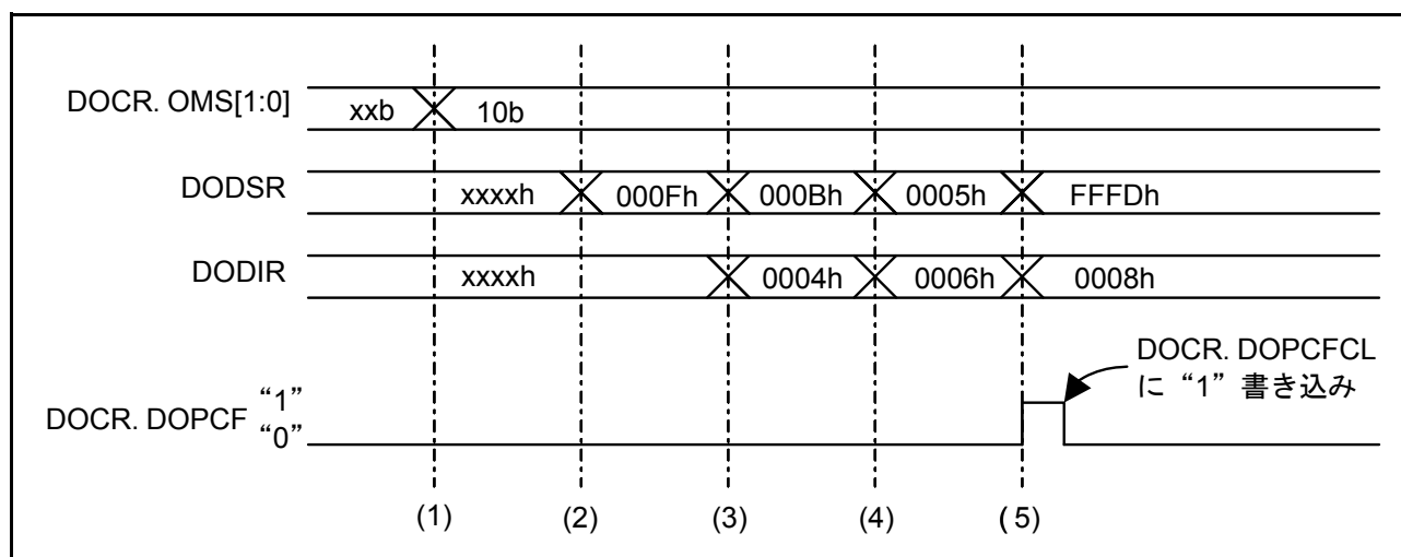
図 40.4 データ減算モードの動作例
