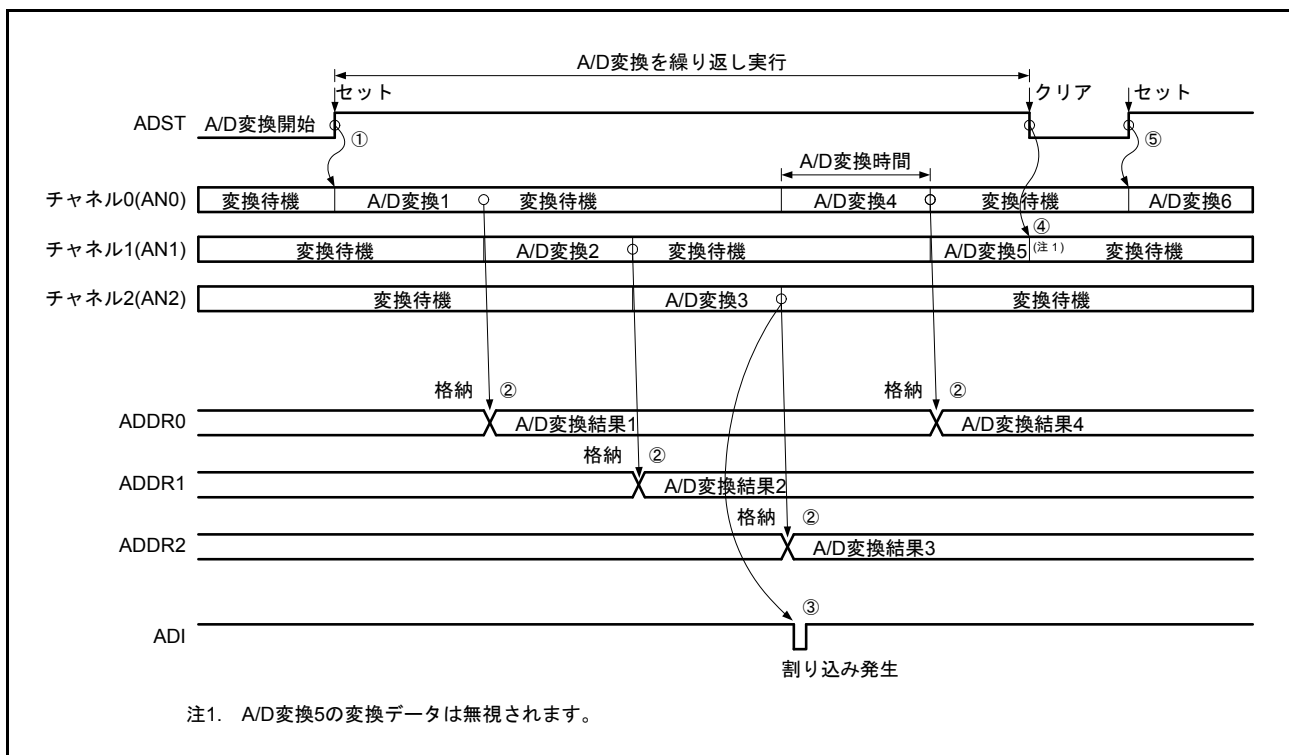
図 35.7 連続スキャンモードの動作例 (基本動作)
