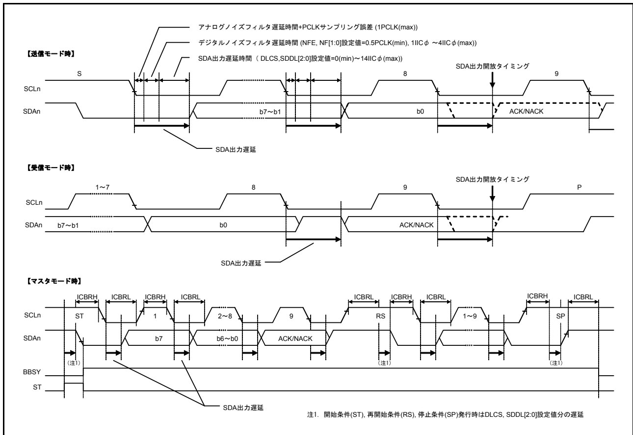
図 31.22 SDA出力遅延タイミング
