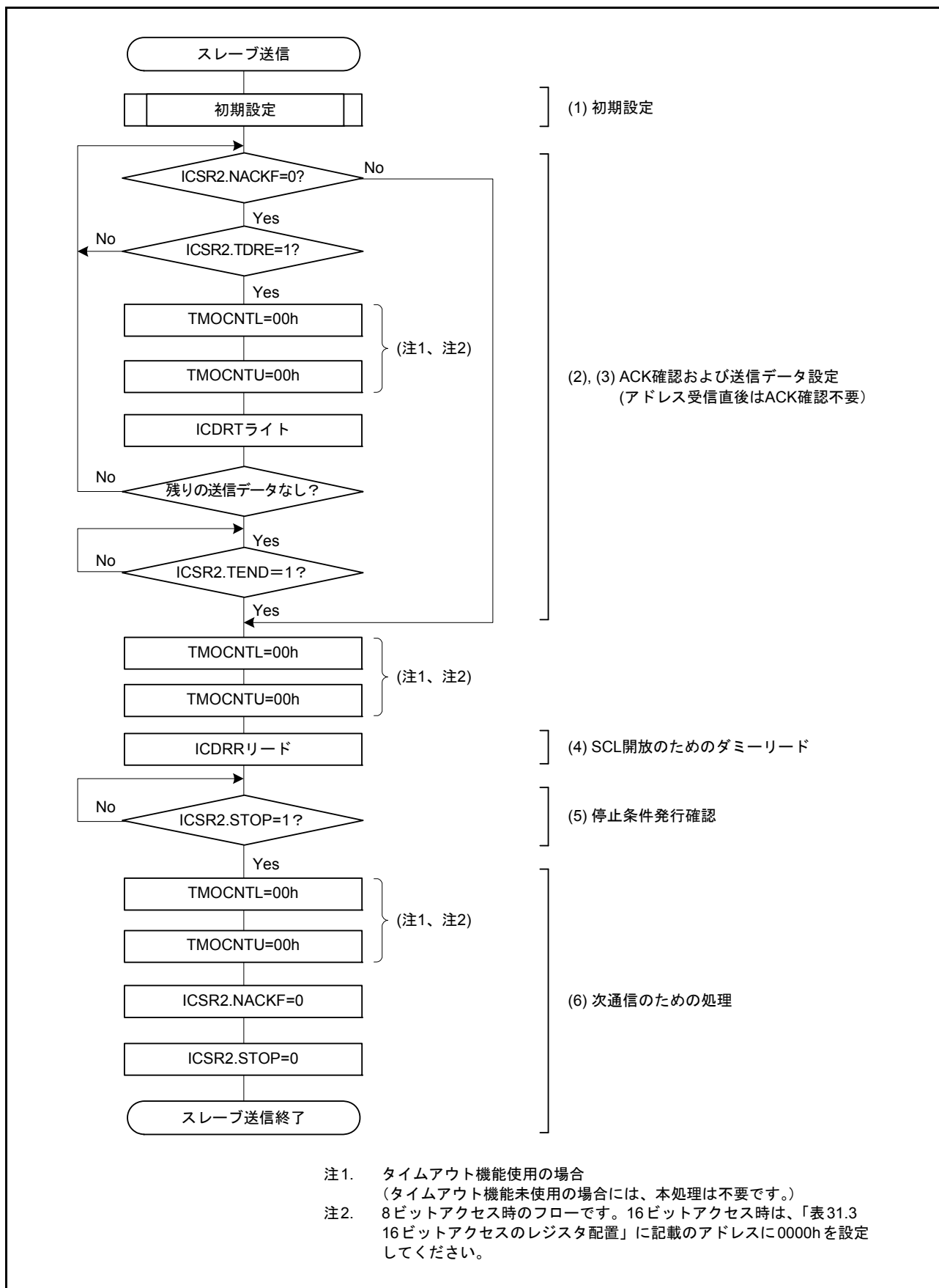
図 31.15 スレーブ送信のフローチャート例
