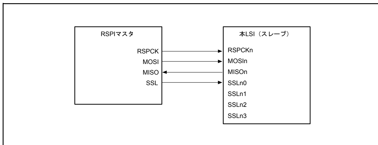
図 32.6 シングルマスタ / シングルスレーブの構成例 (本 LSI = スレーブ、CPHA = 0)
