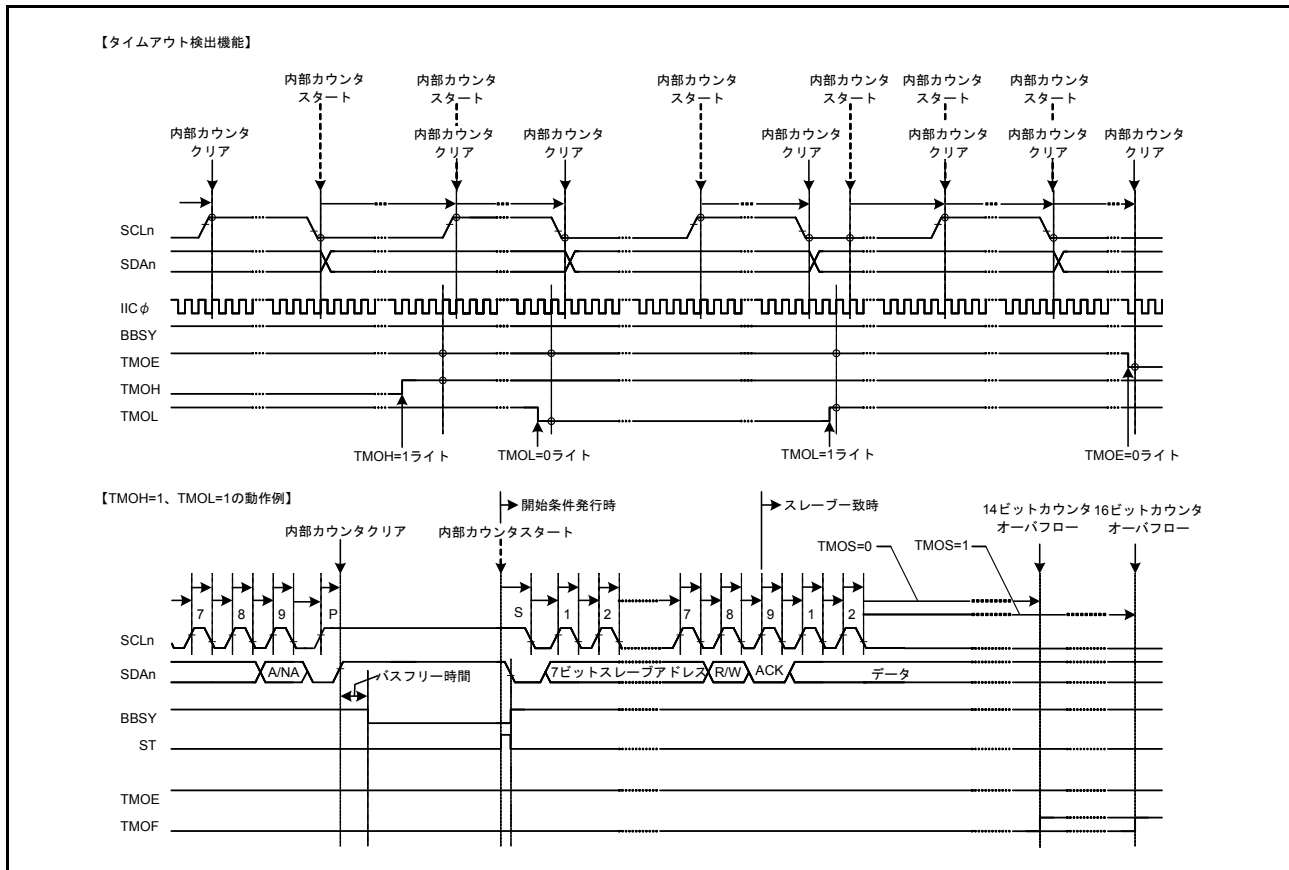
図 31.39 タイムアウト検出機能 (TMOE、TMOS、TMOH、TMOL ビット)
