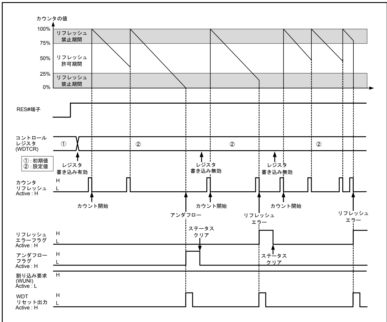
図 27.3 レジスタスタートモード動作例
