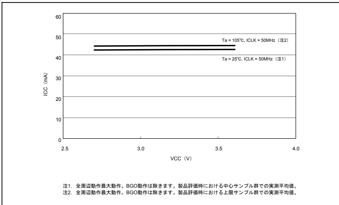
図 44.1 高速動作モードの電圧依存性（参考データ）
