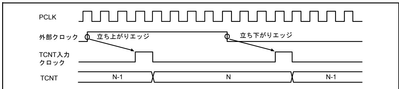
図 22.87 外部クロック動作時のカウントタイミング (位相計数モード)
