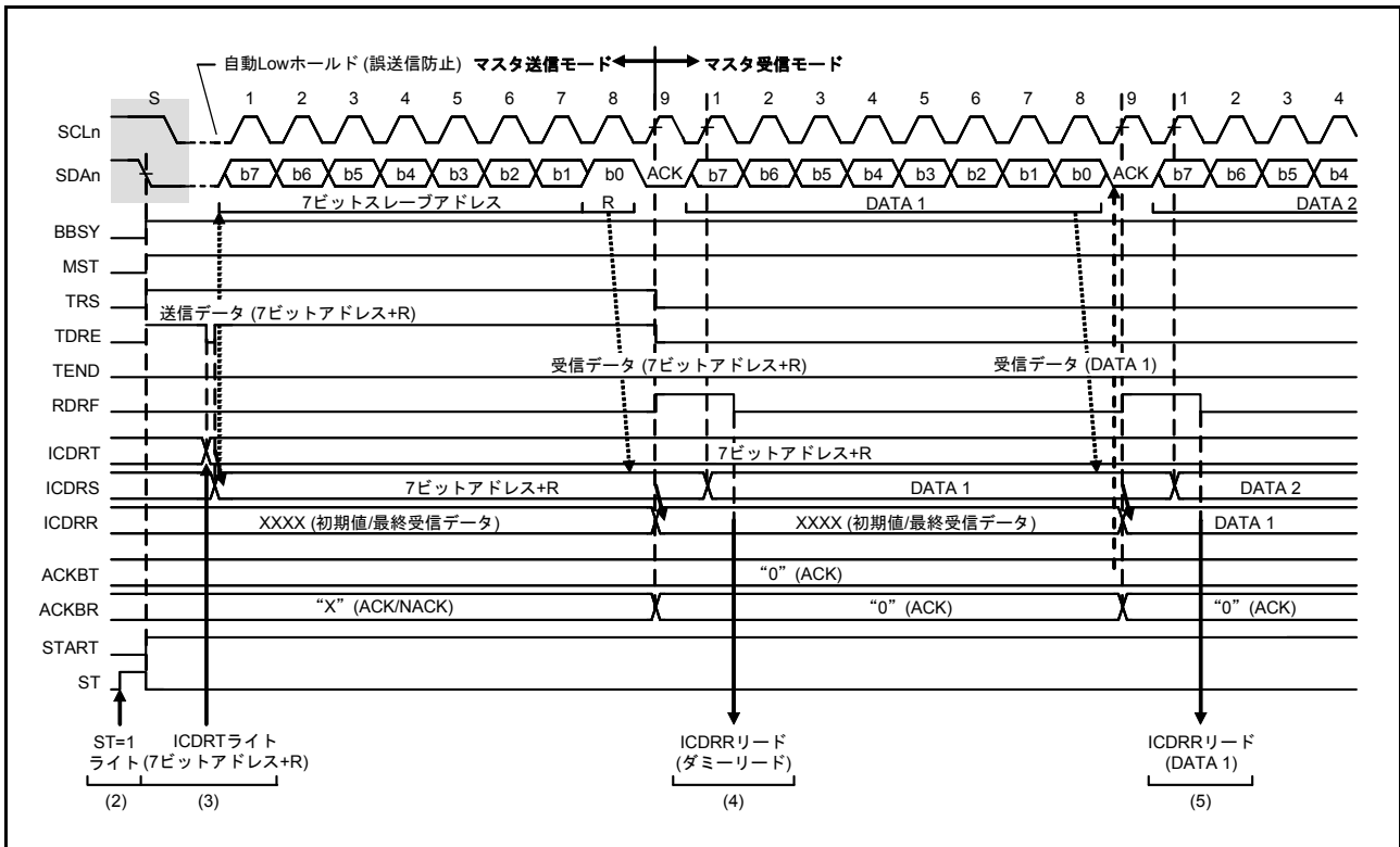
図 31.12 マスタ受信の動作タイミング (1) (7ビットアドレスフォーマット、RDRFS=0 のとき)
