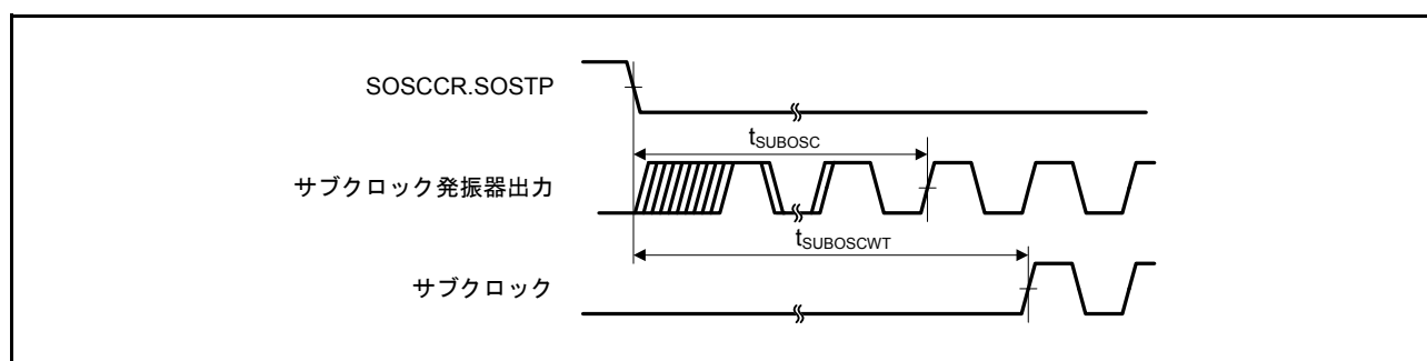
図 44.34 サブクロック発振開始タイミング
