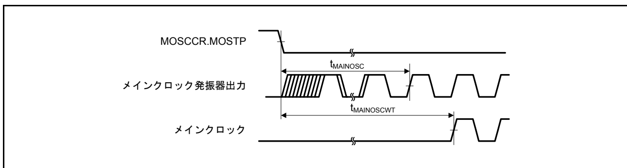
図 44.26 メインクロック発振開始タイミング
