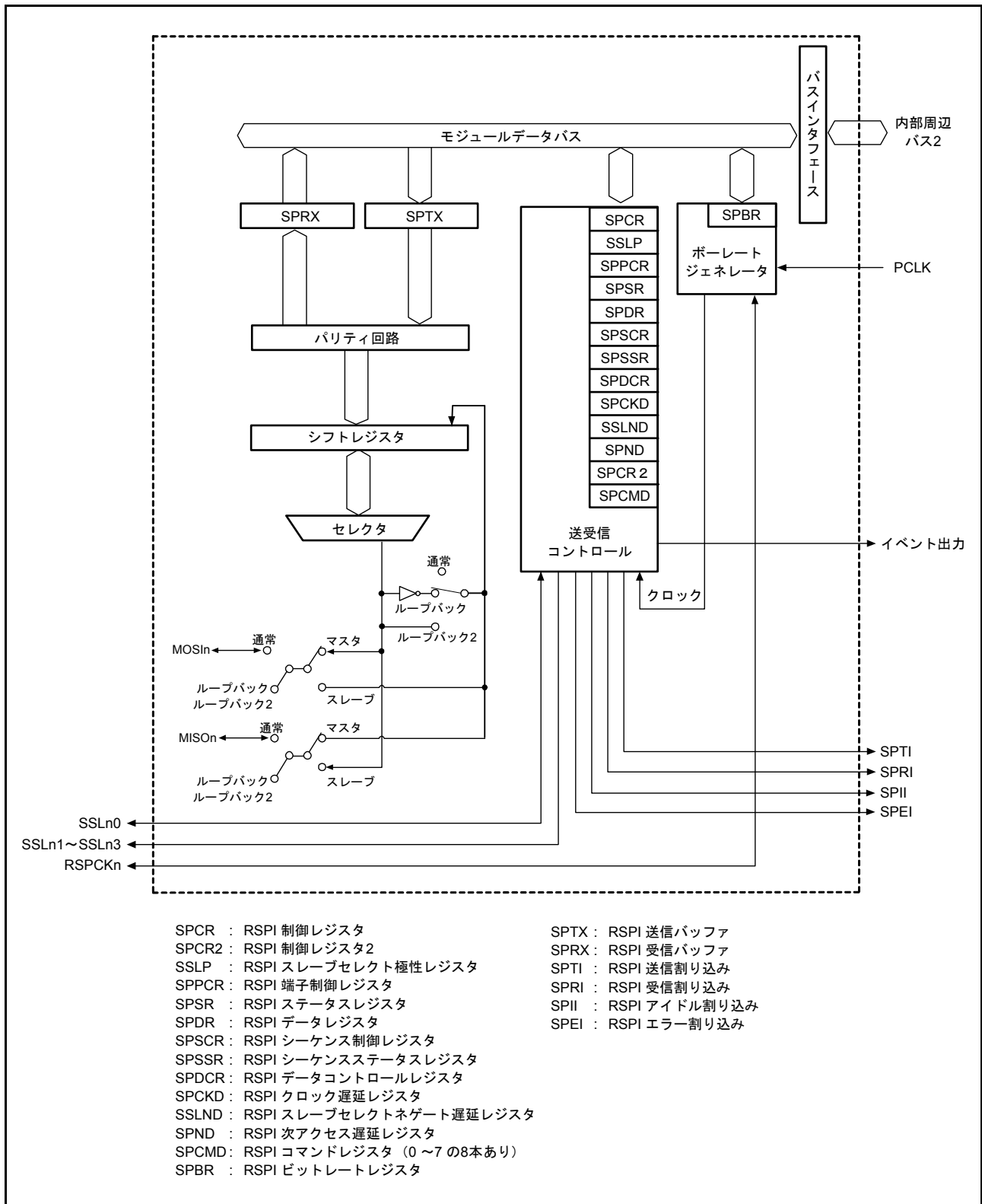
図 32.1 RSPI のブロック図
