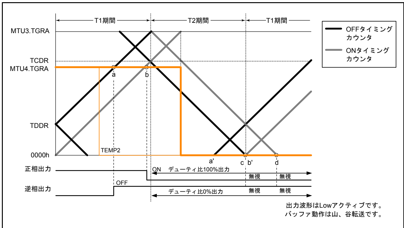
図 22.52 相補 PWM モード 0%、100% 波形出力例 (4)
