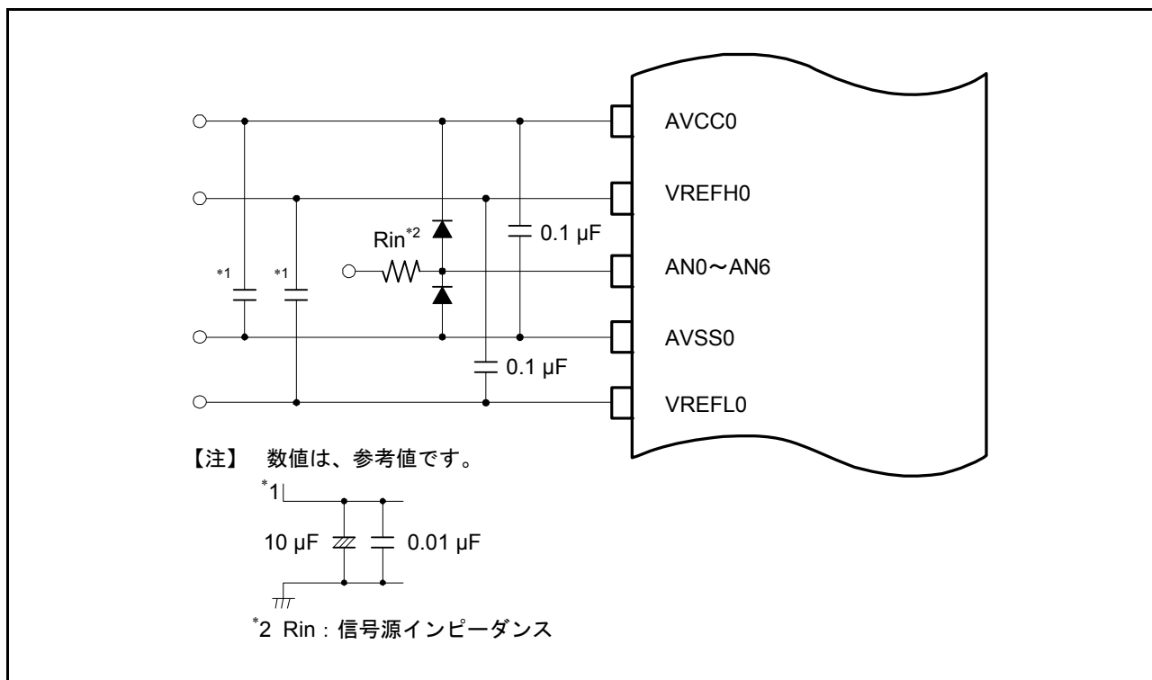
図 35.19 アナログ入力保護回路の例
