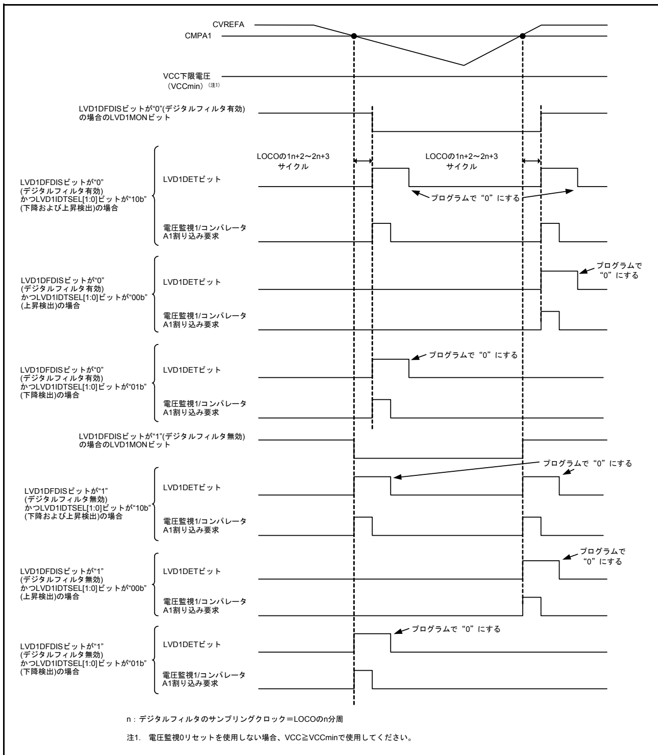
図 38.2 コンパレータ A1 動作例
