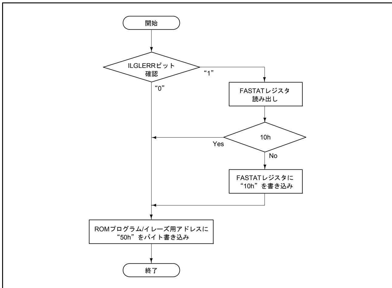
図 42.16 FSTATR0 レジスタのクリア方法
