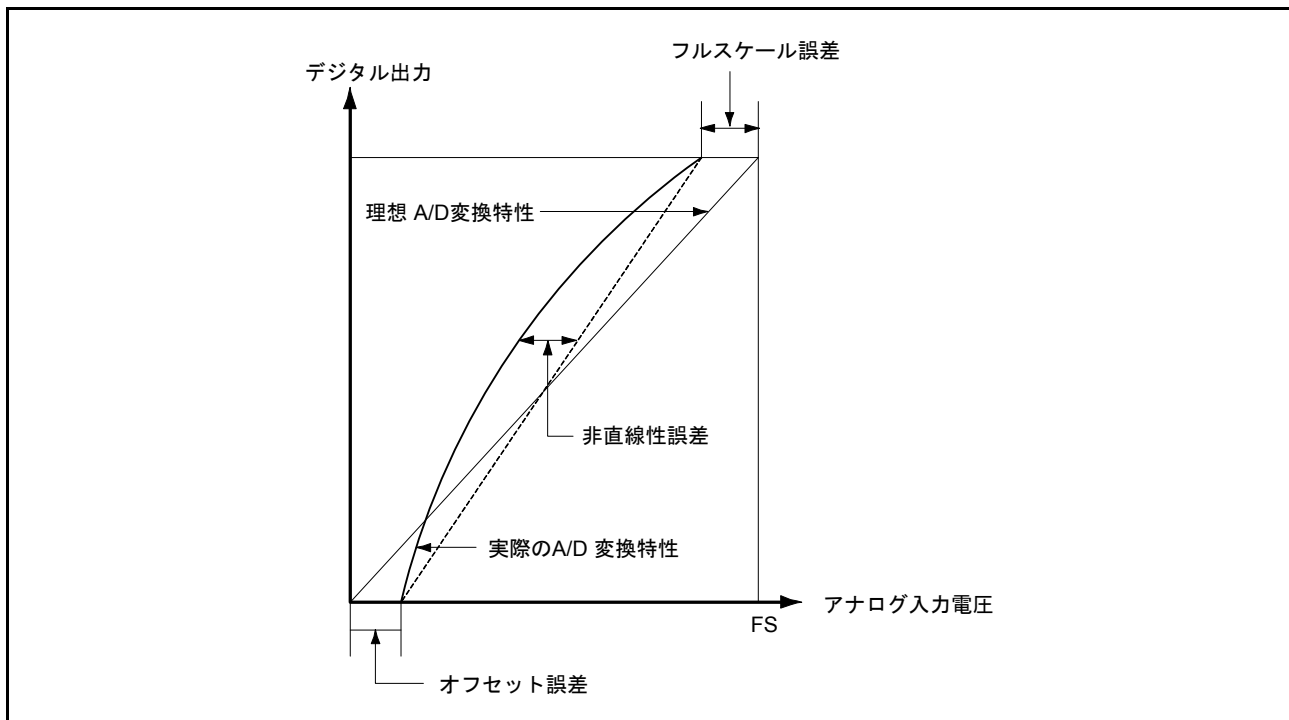
図 35.16 A/D 変換精度の定義 (2)
