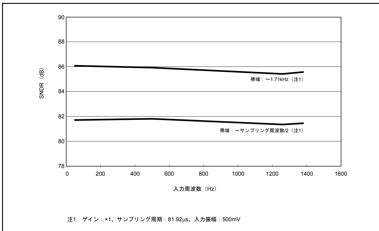
図 44.59 SNDR の入力周波数依存性 (参考データ)
