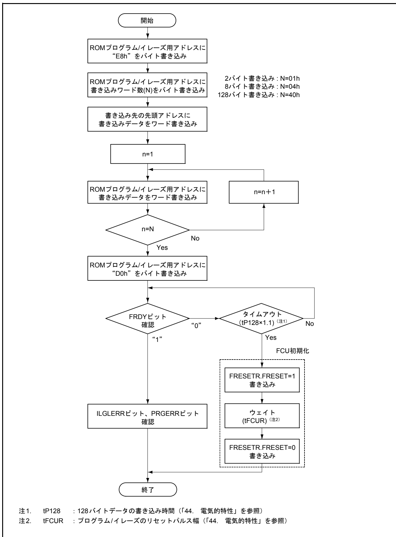
図 42.12 ROM プログラム方法
