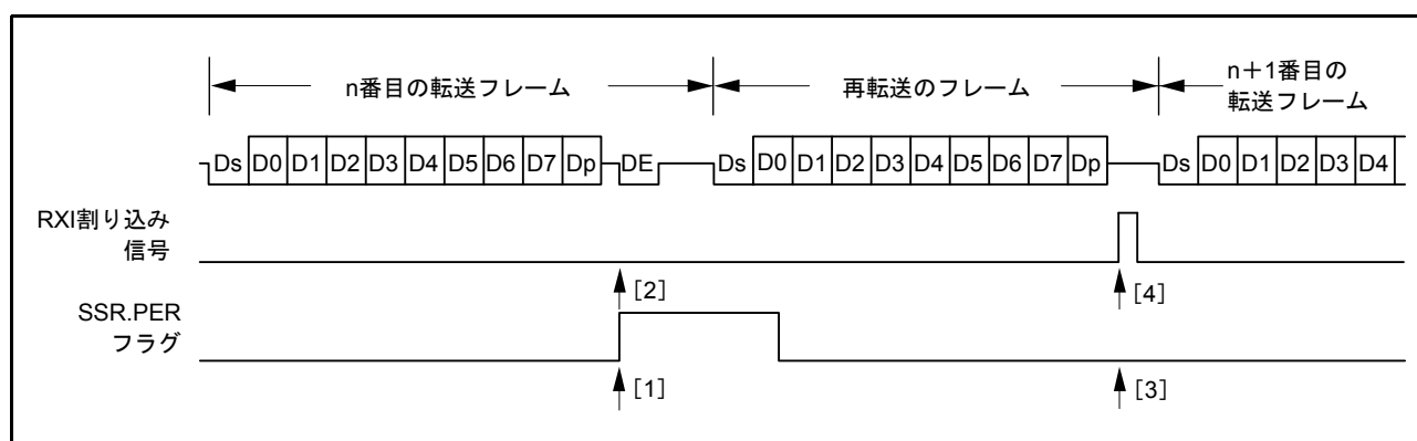
図 29.35 SCI 受信モードの場合の再転送動作（受信時の再転送動作）
