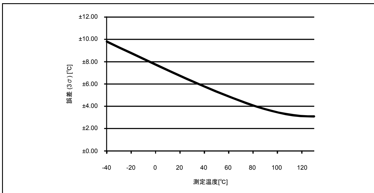
図 37.2 Gバージョン製品の測定誤差 (設計値)
