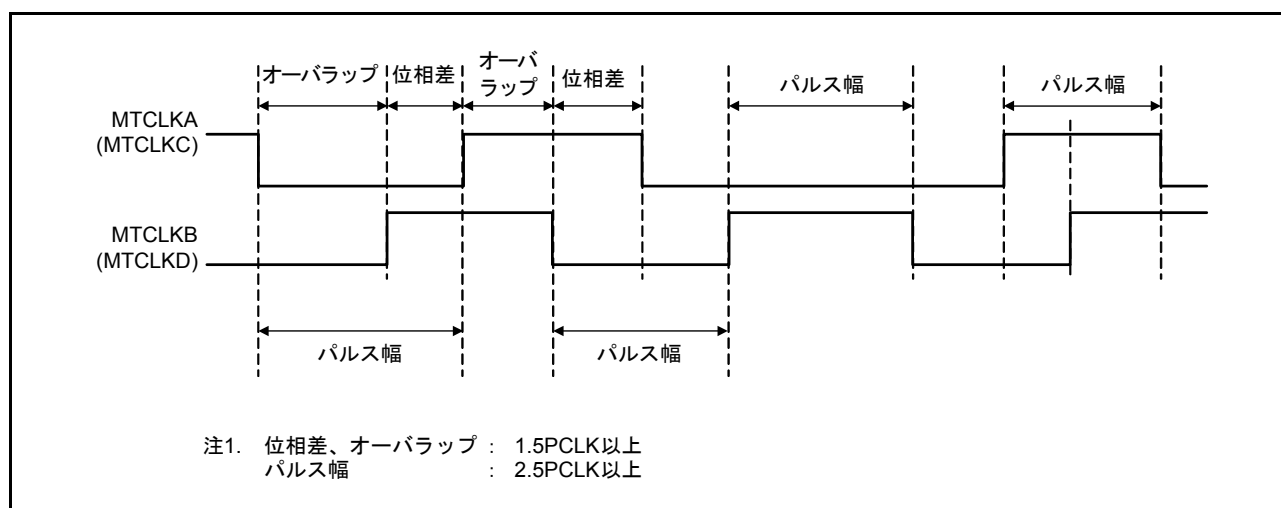
図 22.106 位相計数モード時の位相差、オーバーラップ、およびパルス幅
