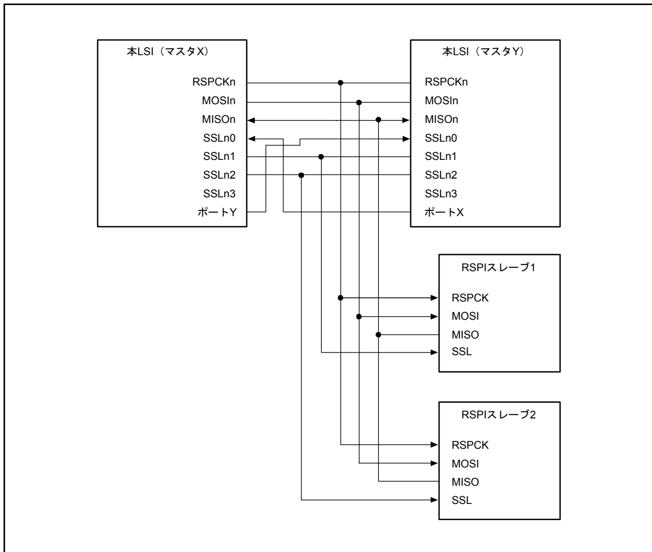
図 32.10 マルチマスタ / マルチスレーブの構成例 (本 LSI = マスタ)
