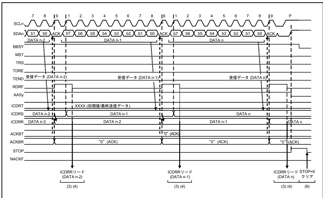
図 31.20 スレーブ受信の動作タイミング (2) (RDRFS=0 のとき)
