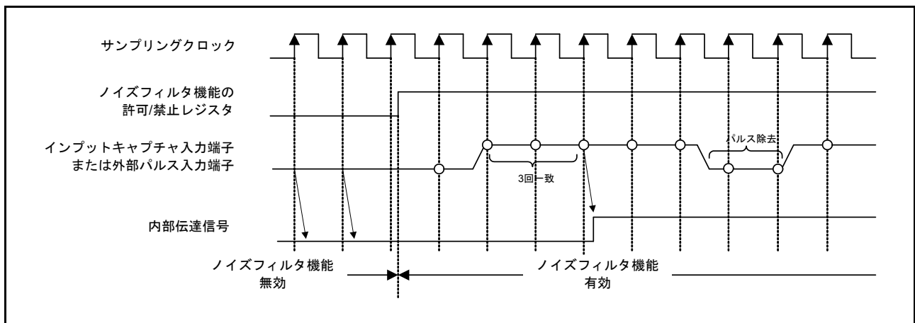
図 22.83 ノイズフィルタのタイミング
