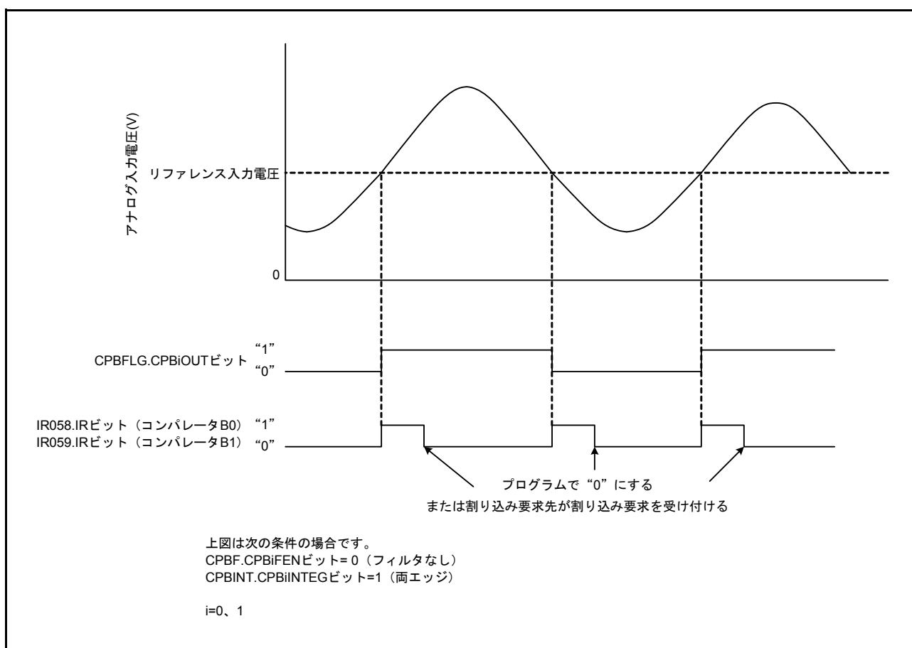
図 39.2 コンパレータ Bi (i = 0、1) の動作例
