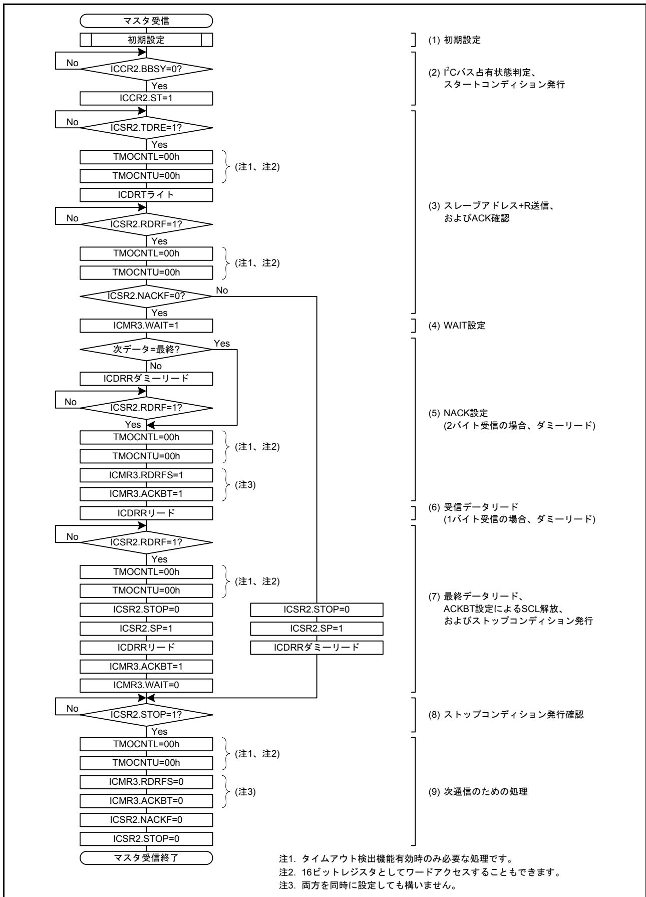
図 31.10 マスタ受信のフローチャート例 (7ビットアドレスフォーマットの場合、2バイト以下の場合)
