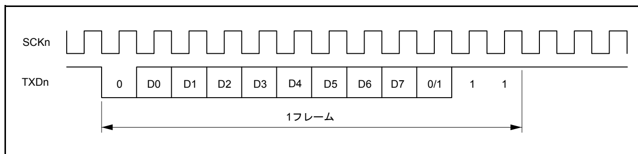
図 29.6 出カクロックと送信データの位相関係（調歩同期式モード：SMR.CHR=0,PE=1,MP=0,STOP=1）
