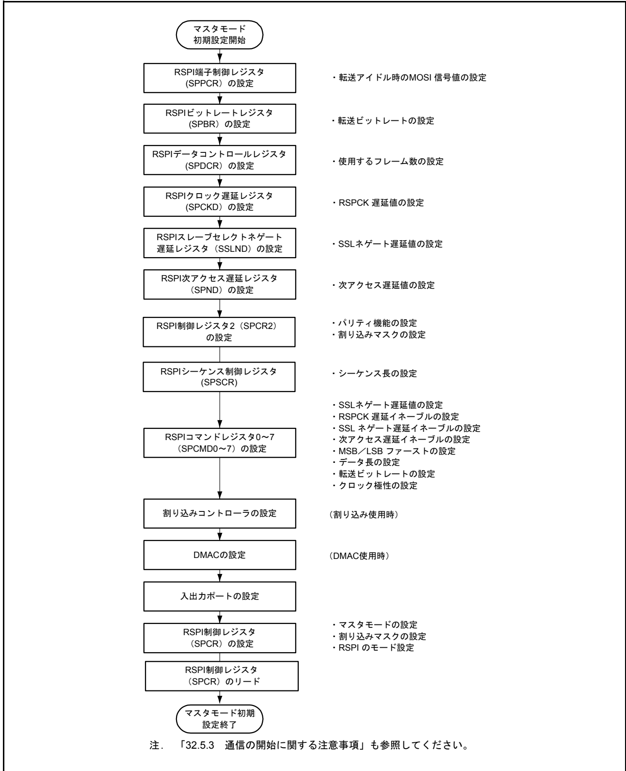
図 32.45 マスターモード時の初期化フロー例 (クロック同期式動作)
