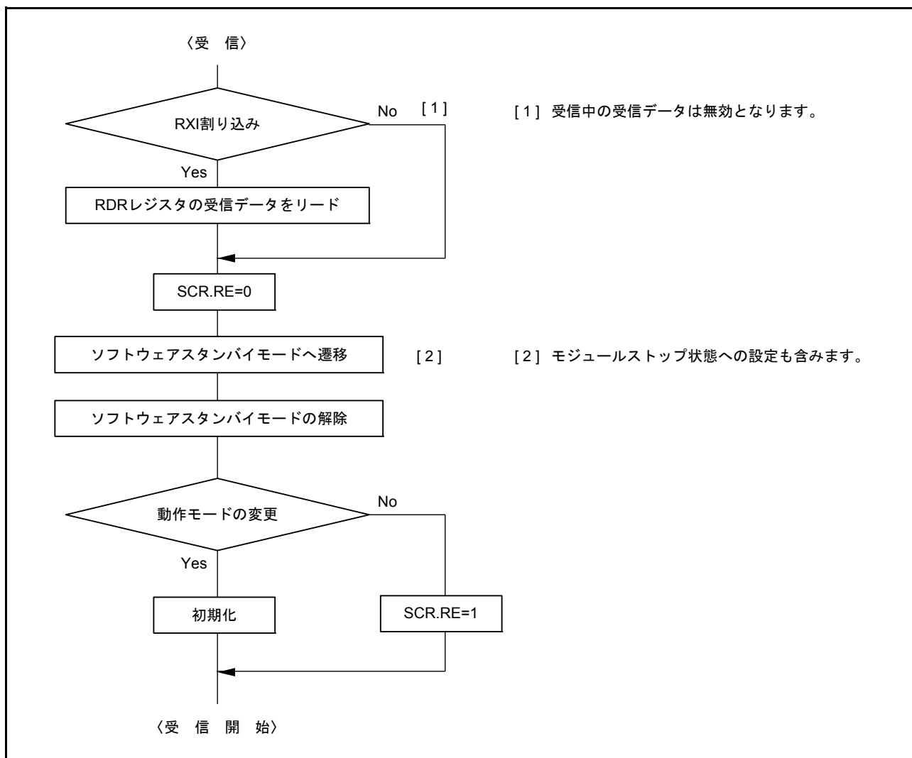
図 29.56 受信時のソフトウェアスタンバイモード遷移フローチャートの例
