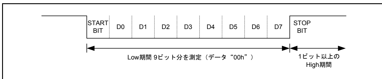
図 42.23 ビットレート自動調整時の SCI 送受信フォーマット
