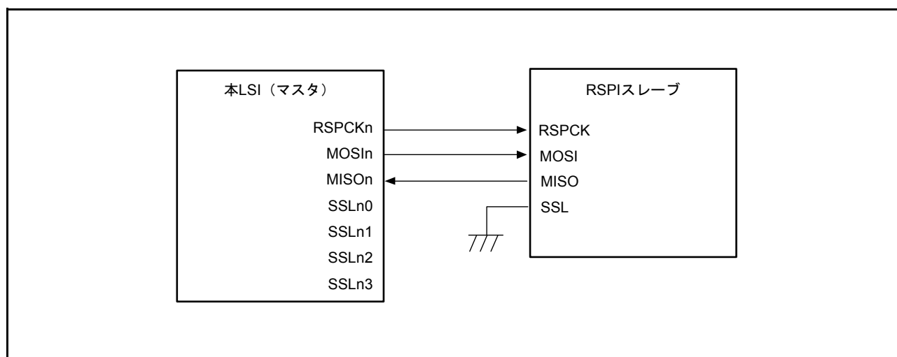
図 32.5 シングルマスタ / シングルスレーブの構成例 (本 LSI = マスタ)
