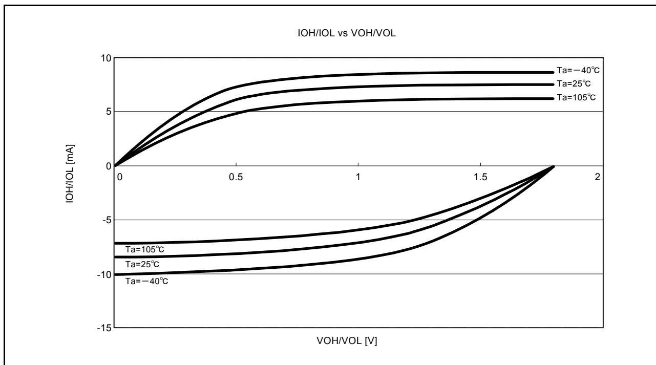
図 44.17 高駆動出力を選択したときの VOH/VOL IOH/IOL 温度特性 VCC = 1.8V (参考データ)
