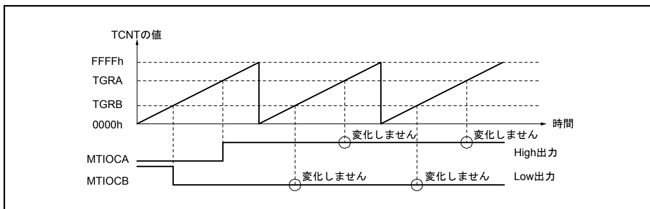
図 22.8 Low 出力/High 出力の動作例
