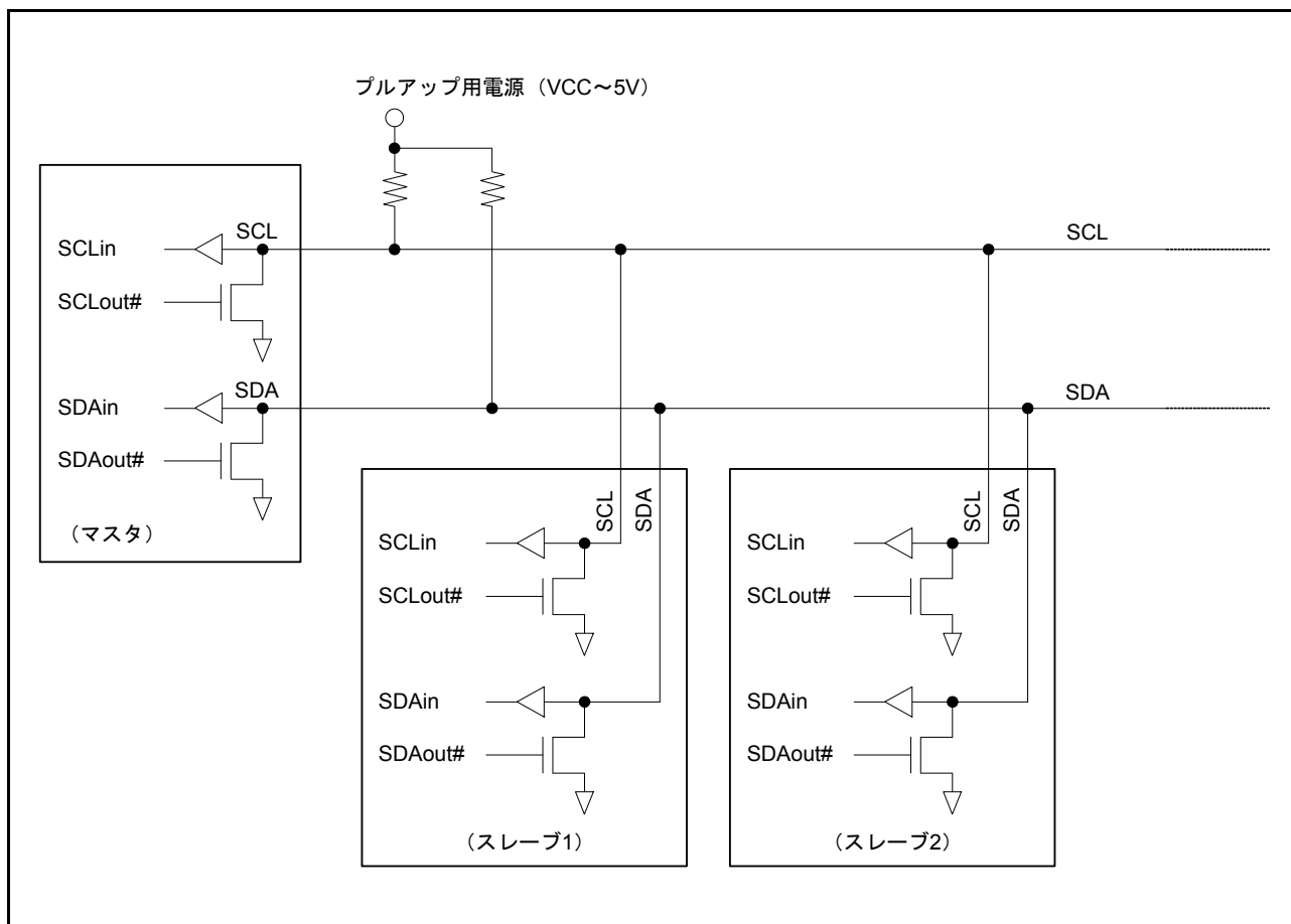
図 31.2 入出力端子の外部回路接続例 (I 2 C バス構成例)
