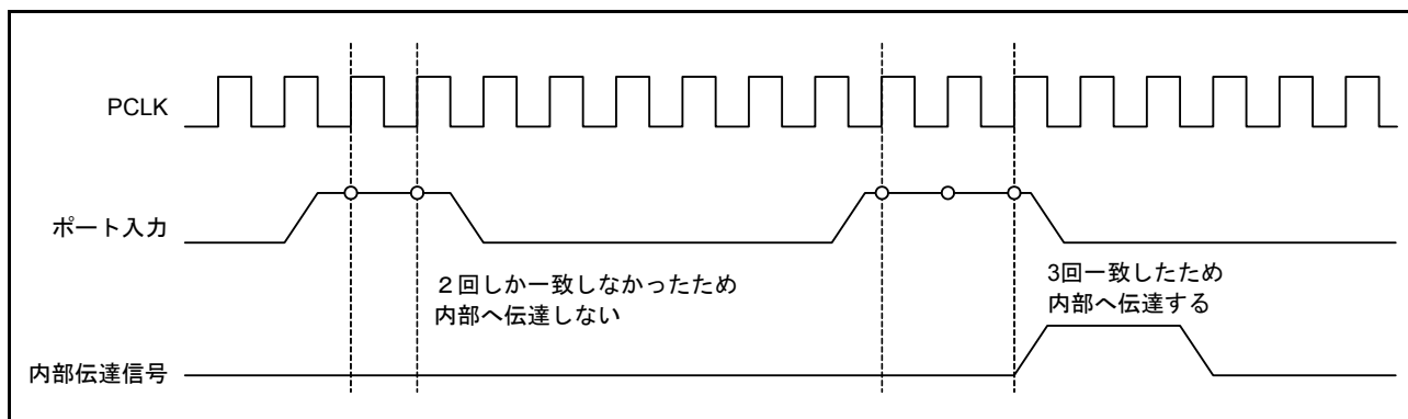
図 19.7 ポート入力のデジタルフィルタの動作
