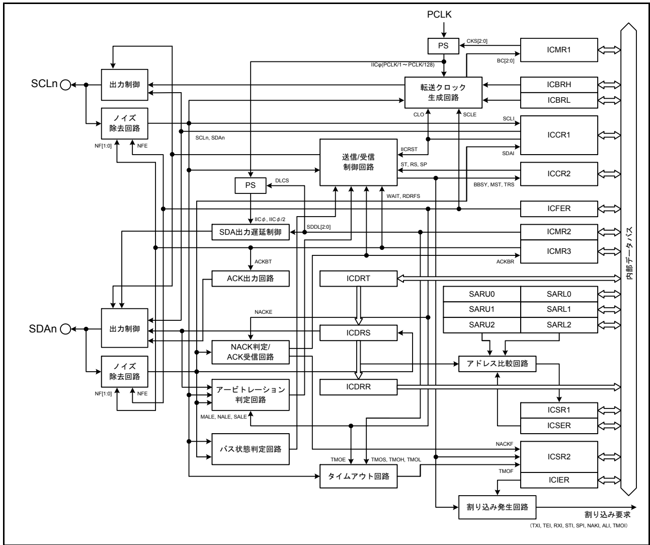
図 31.1 RIIC のブロック図
