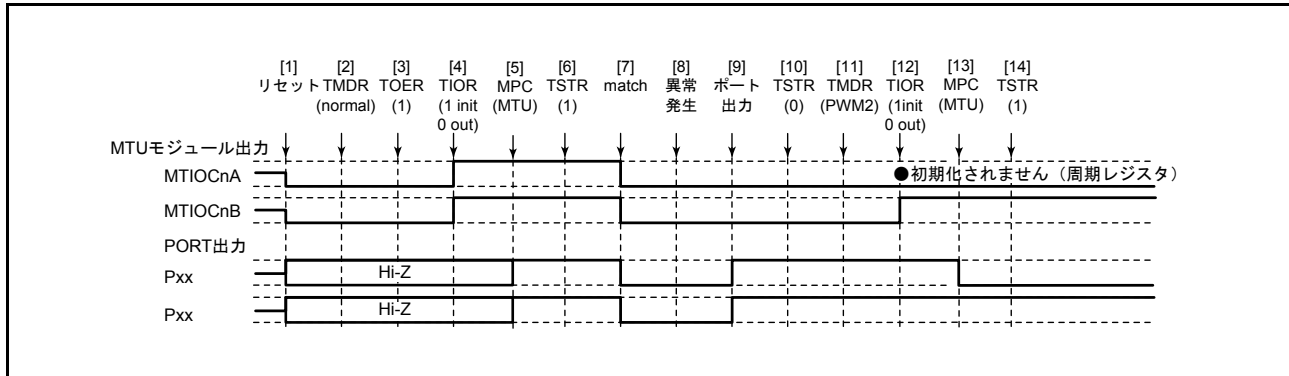
図 22.127 ノーマルモードで異常が発生し、PWM モード2で復帰する場合
