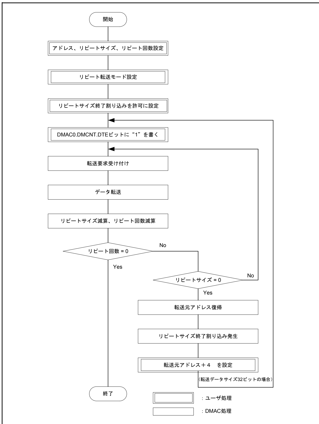
図 17.9 リPEAT転送モード + オフセット加算による XY 変換のフロー
