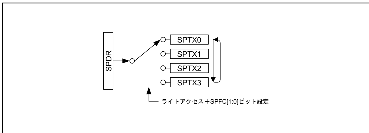
図 32.3 SPDR レジスタの構成図 (ライト時)
