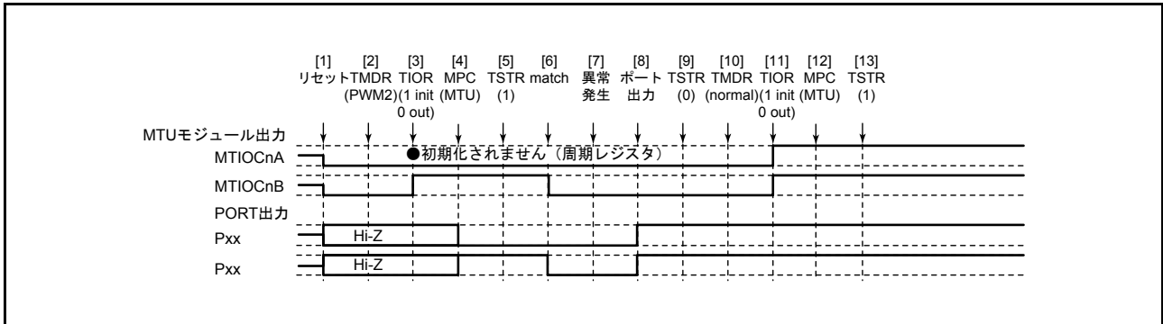
図 22.137 PWM モード 2 で異常が発生し、ノーマルモードで復帰する場合
