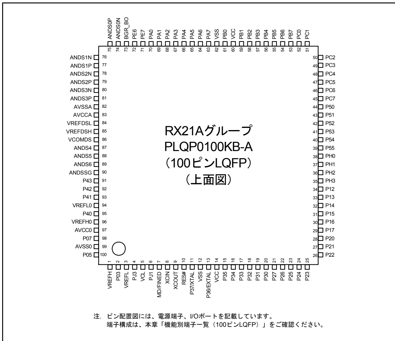
図 1.3 100 ピン LQFP ピン配置図
