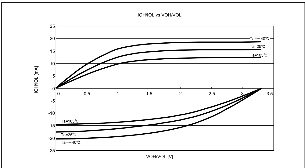
図 44.14 通常出力を選択したときの VOH/VOL IOH/IOL 温度特性 VCC = 3.3V (参考データ)
