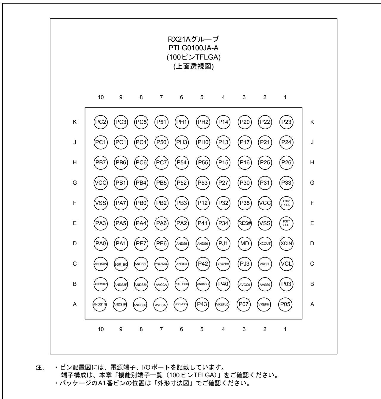
図 1.6 100ピン TFLGA ピン配置図（上面透視図）
