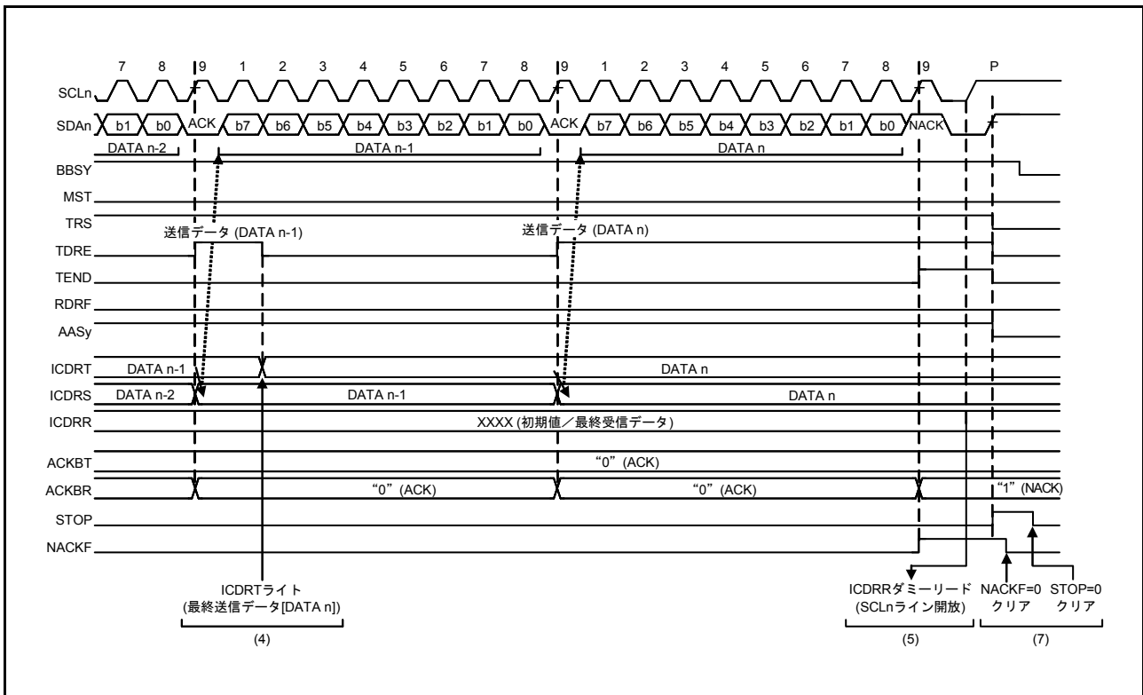
図 31.17 スレーブ送信の動作タイミング (2)
