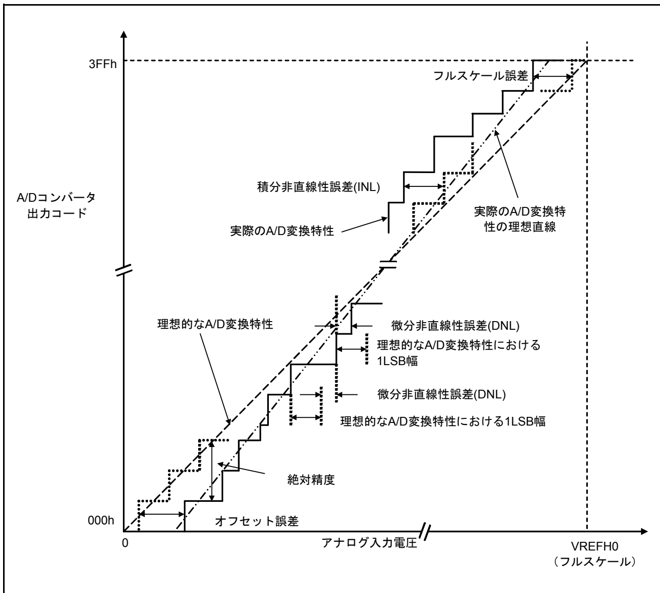
図 44.62 A/D コンバータ特性用語説明図
