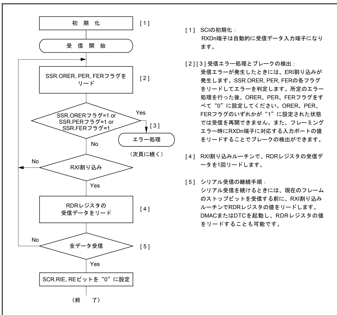
図 29.12 調歩同期式モードのシリアル受信のフローチャート例 (1)
