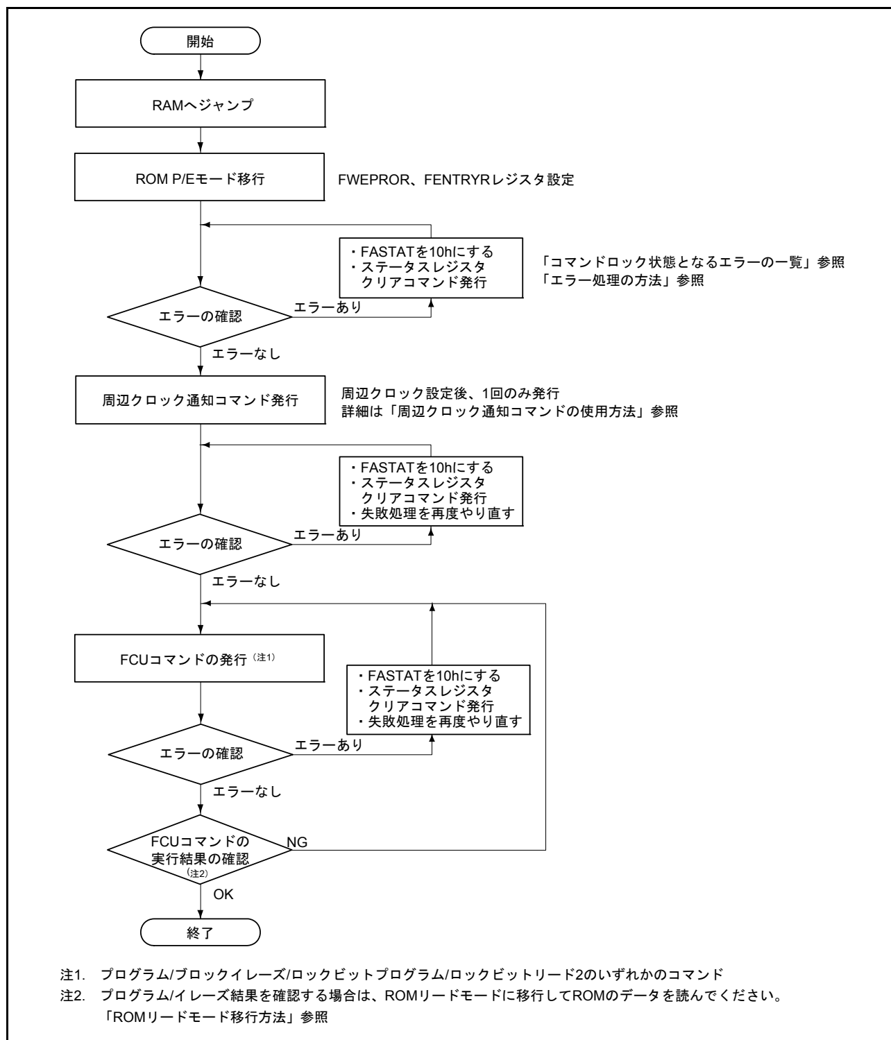
図 42.10 プログラム/イレーズ処理の概略フロー
