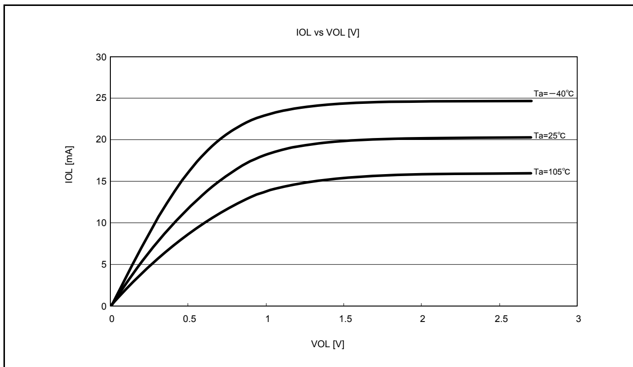
図 44.22 RIIC 出力端子の VOL、IOL 温度特性 VCC = 2.7V (参考データ)
