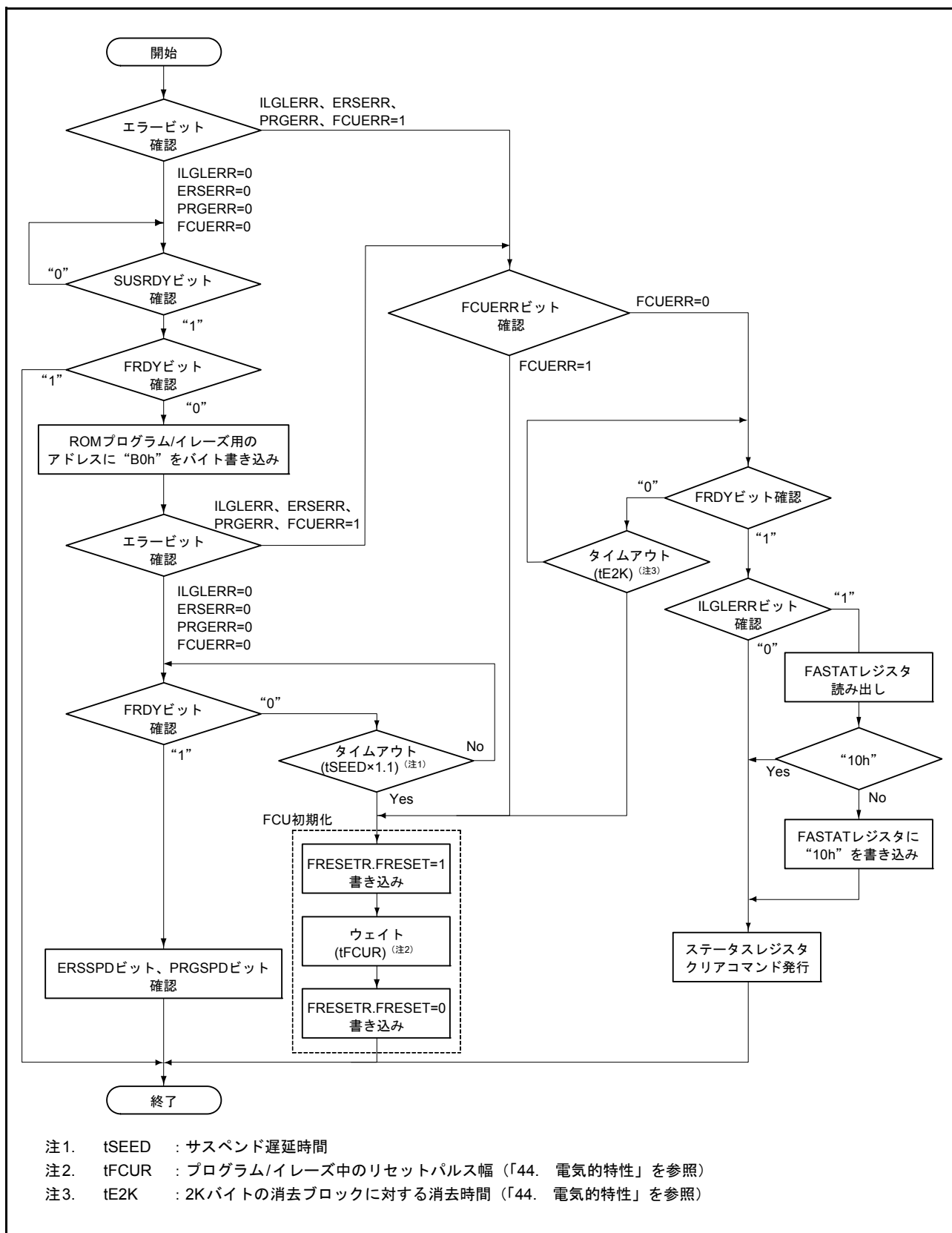
図 42.17 プログラム/イレーズのサスペンド方法
