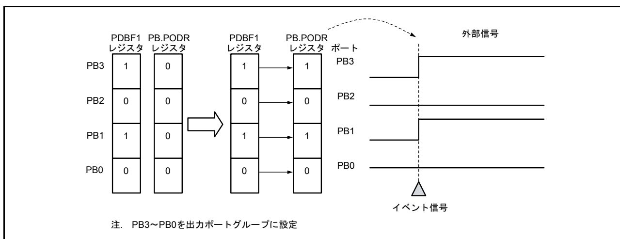
図 19.5 出力ポートグループのイベントリンク動作
