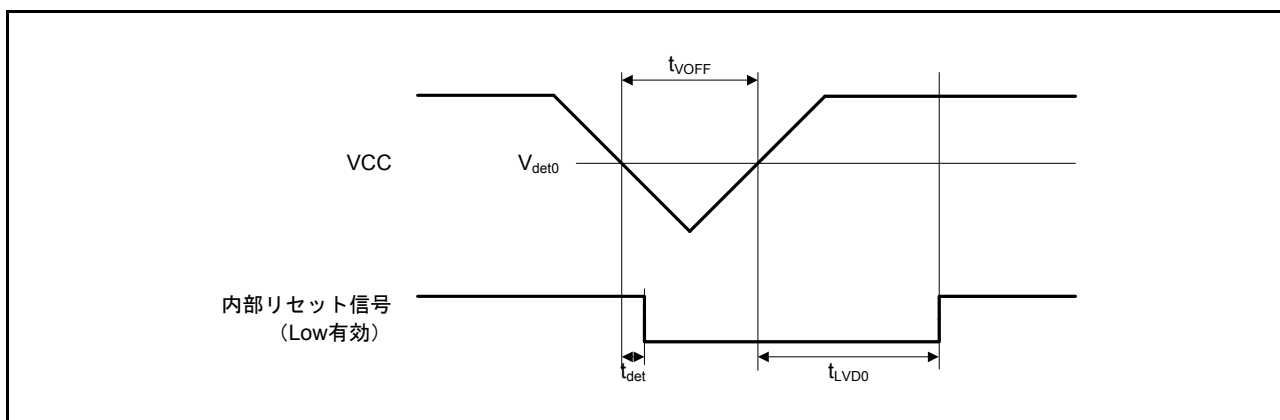
図 44.66 電圧検出回路タイミング (V det0 )
