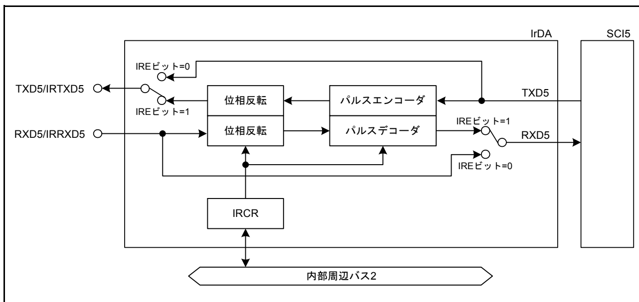
図 30.1 IrDA と SCI5 の連携イメージのブロック図
