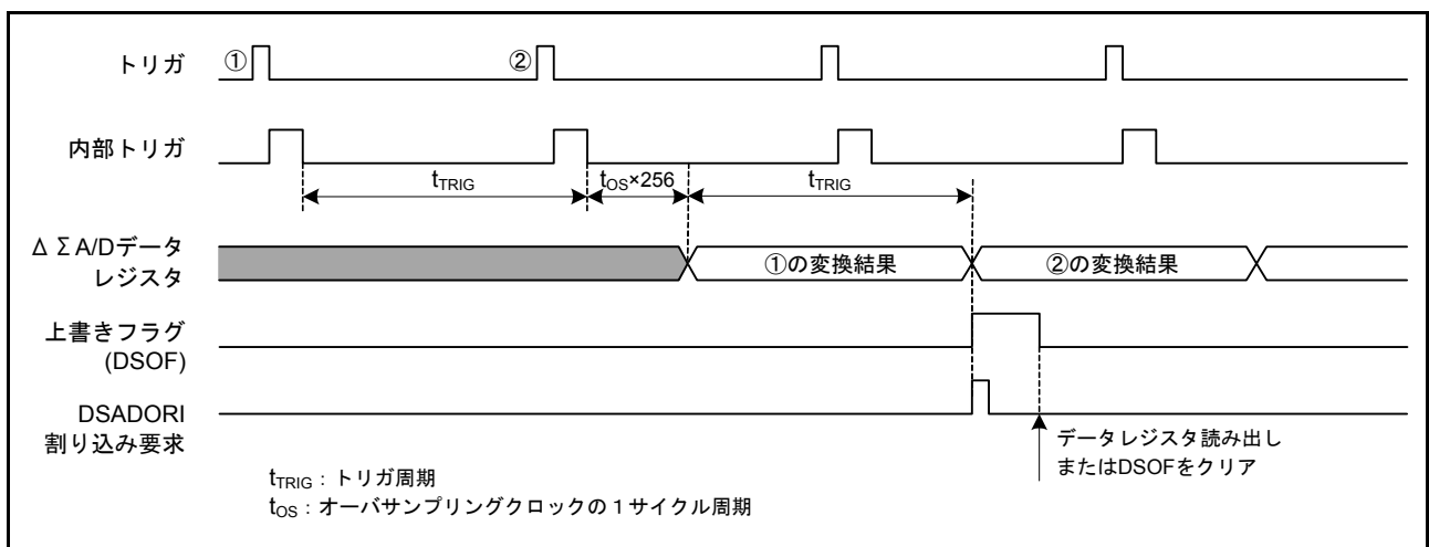
図 34.7 データレジスタ上書き発生時の動作例
