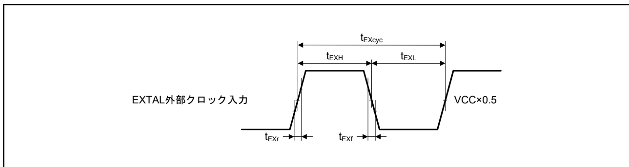
図 44.25 EXTERNAL クロック入力タイミング
