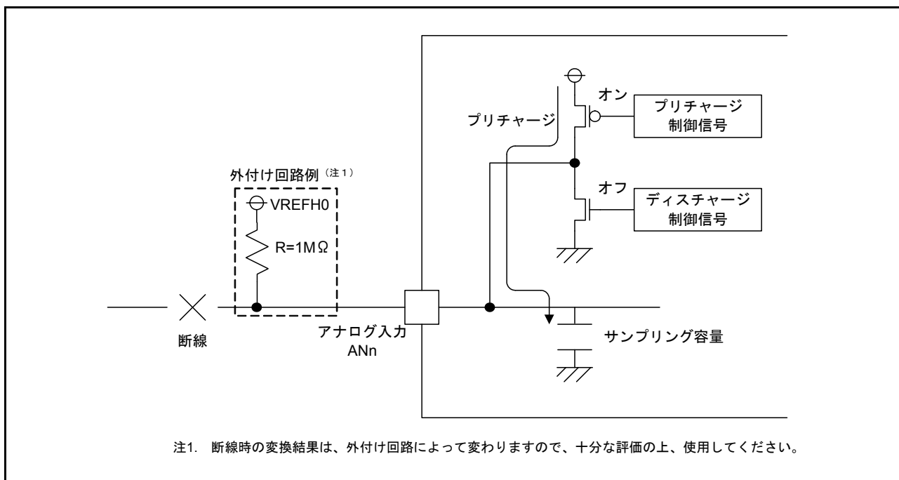
図 35.12 VREFH0 側での断線検出例 (プリチャージを選択)
