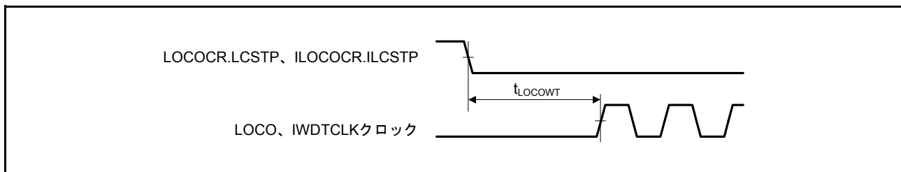
図 44.27 LOCO、IWDTCLK クロック発振開始タイミング
