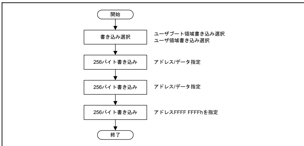
図 42.28 ブートモードでのROM 書き込み方法
