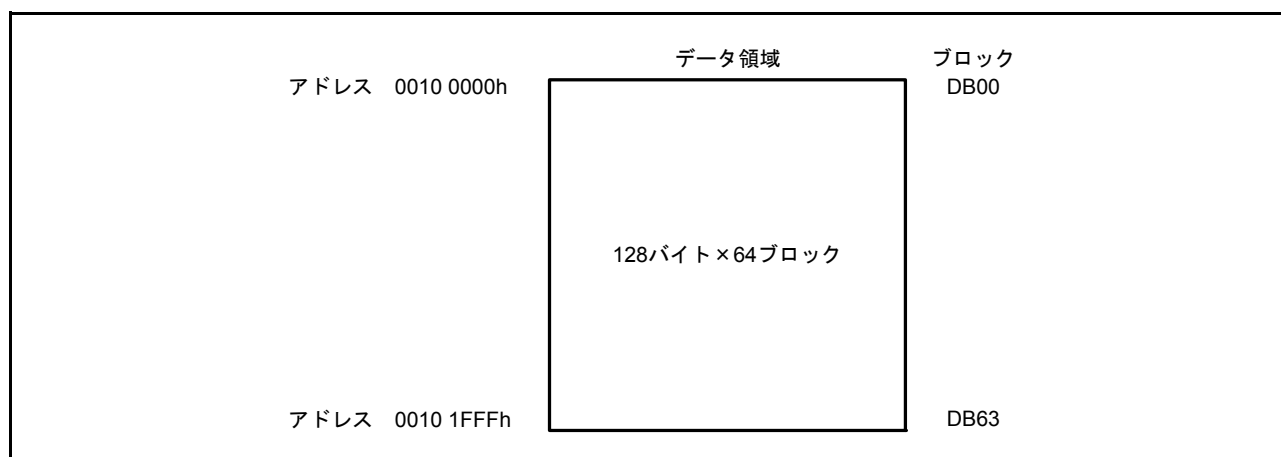
図 43.3 データ領域のブロック分割
