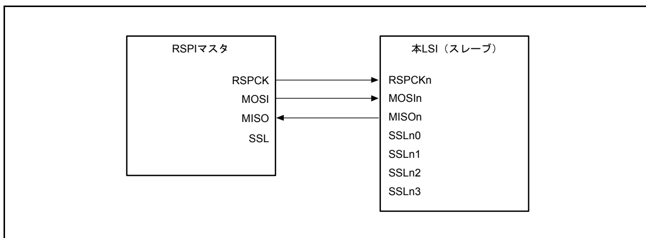
図 32.12 マスタ (クロック同期式動作) / スレーブ (クロック同期式動作) の構成例 (本 LSI = スレーブ、CPHA = 1)
