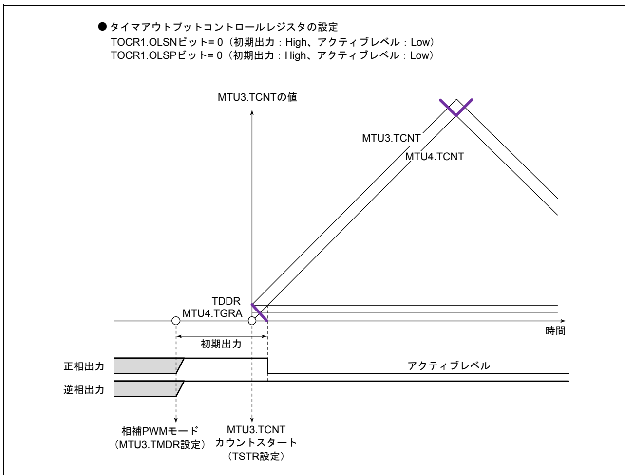
図 22.45 相補 PWM モードの初期出力例 (2)
