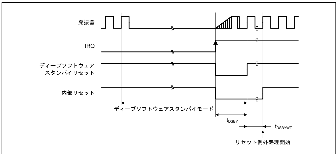
図 44.38 ディープソフトウェアスタンバイモード解除タイミング
