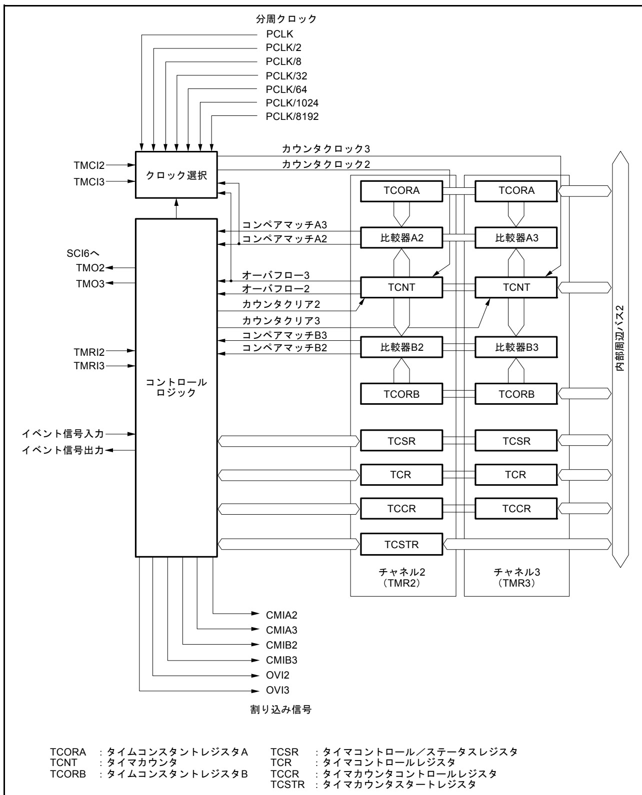
図 24.2 TMR (ユニット 1) のブロック図
