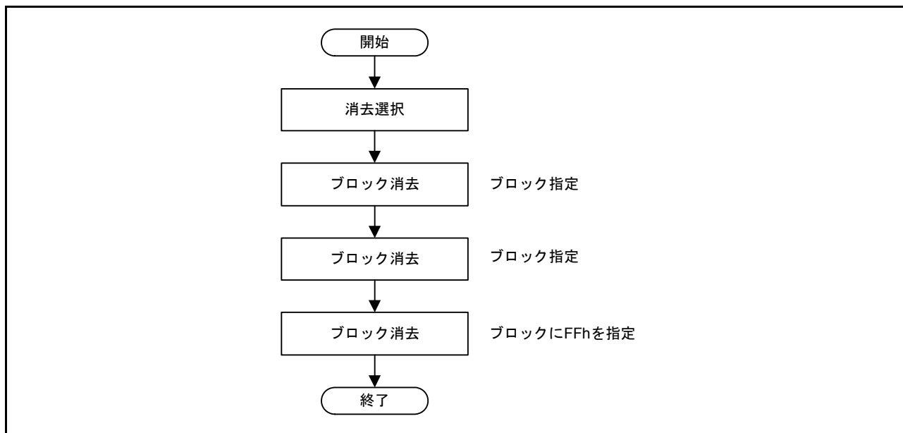
図 42.29 ブートモードでのROM 消去方法
