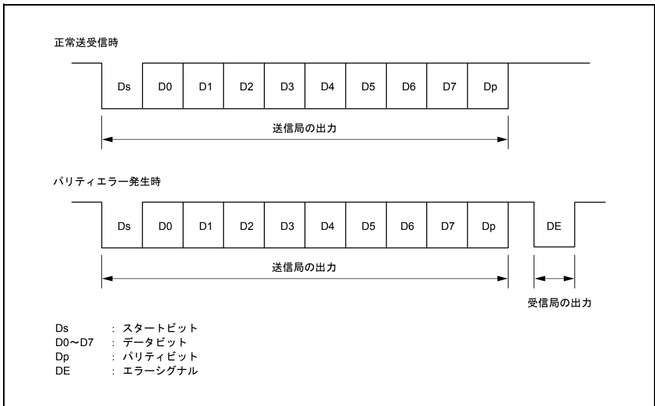
図 29.28 スマートカードインタフェースモードのデータフォーマット
