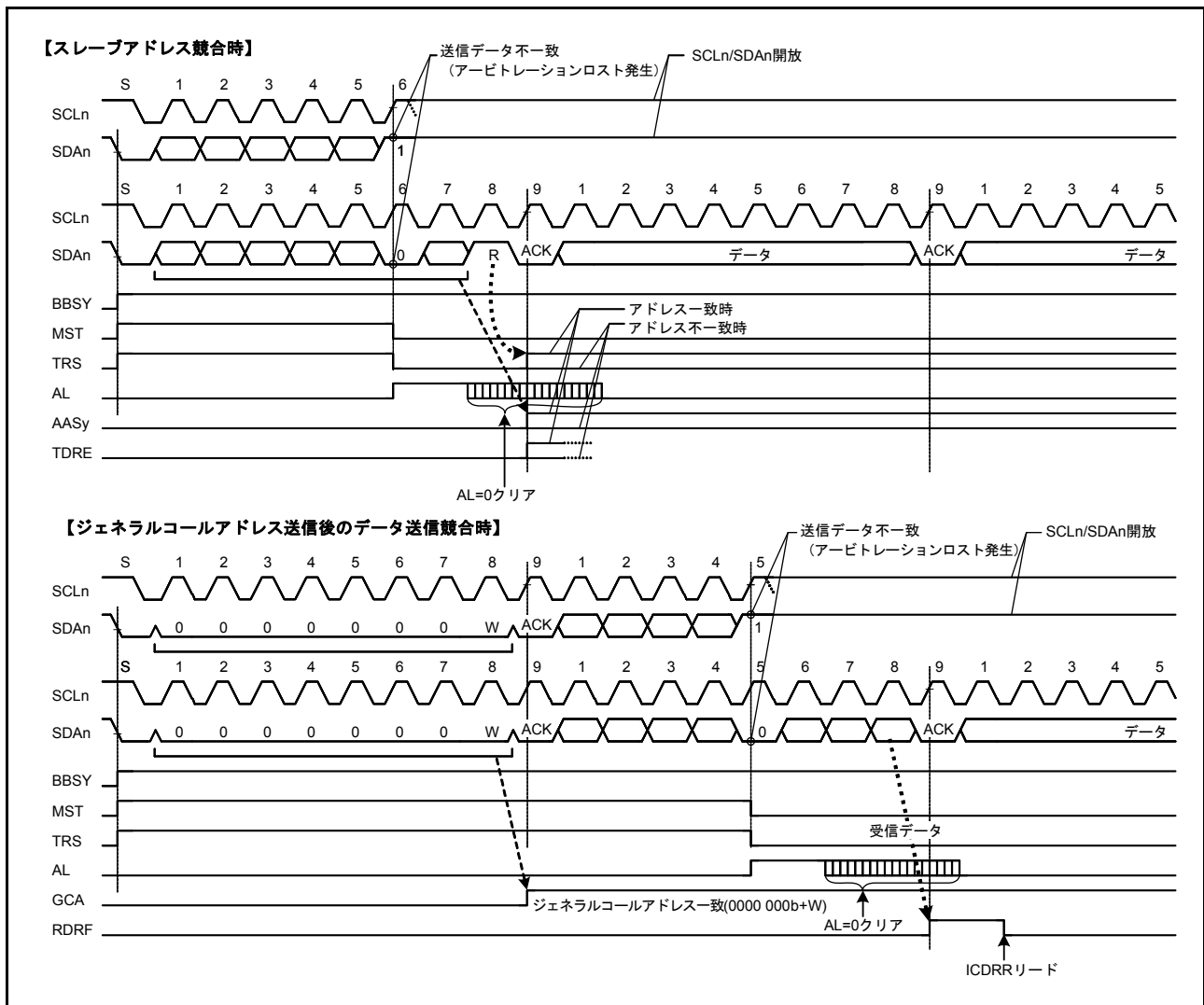
図 31.33 マスタアービトレーションロスト検出動作例 (MALE=1 のとき)
