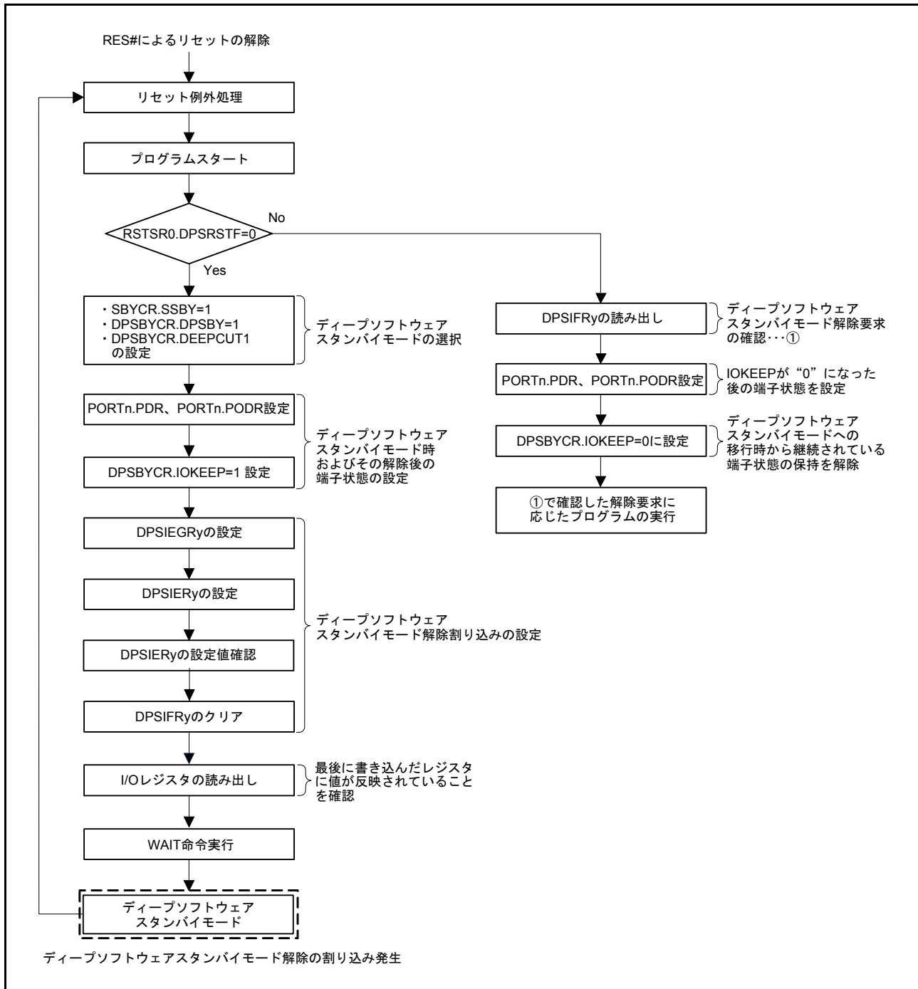
図 11.9 ディープソフトウェアスタンバイモードのフローチャート例
