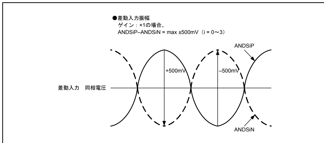
図 44.55 差動入力振幅
