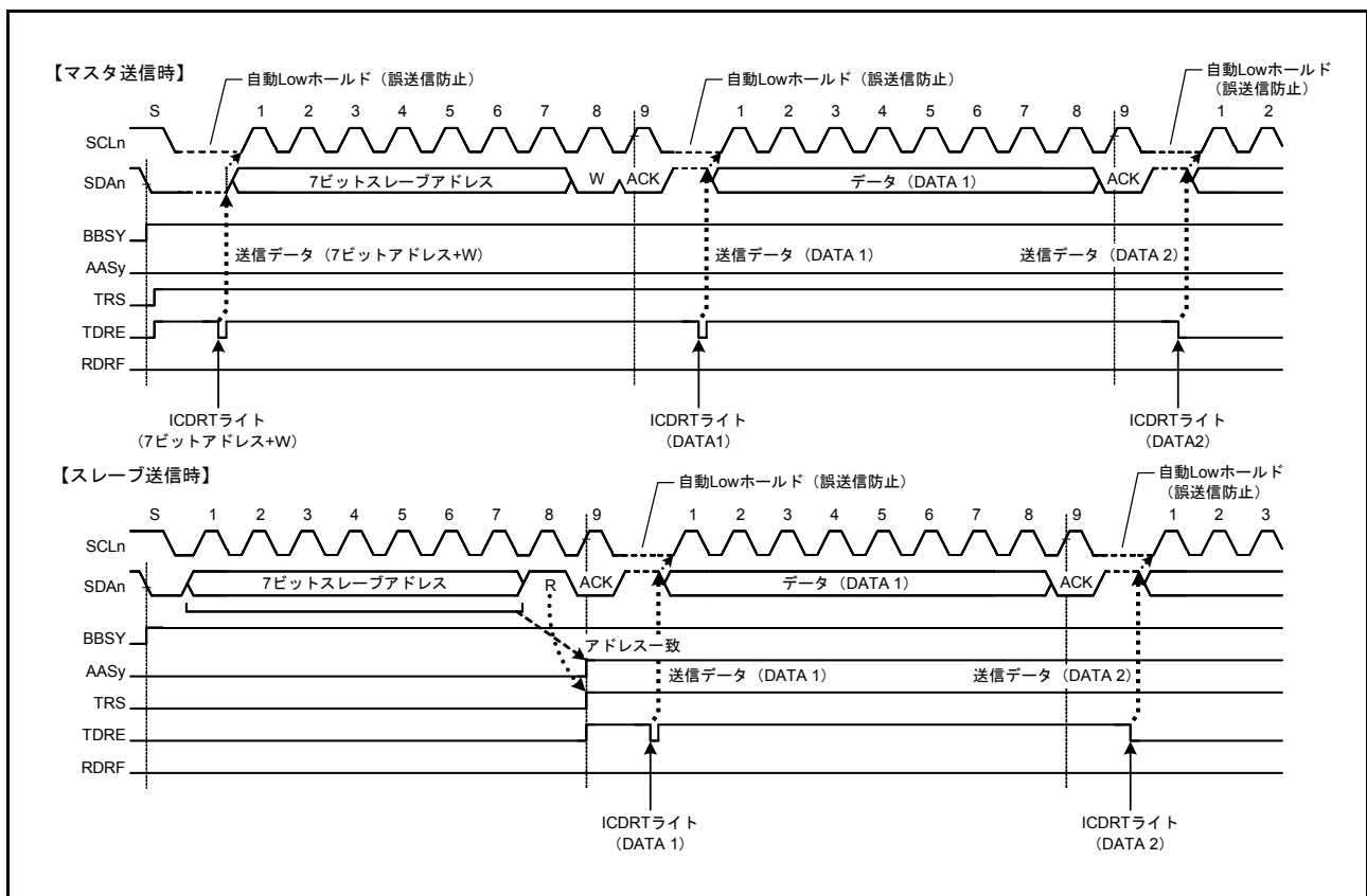
図 31.30 送信モードの自動 Low ホールド動作
