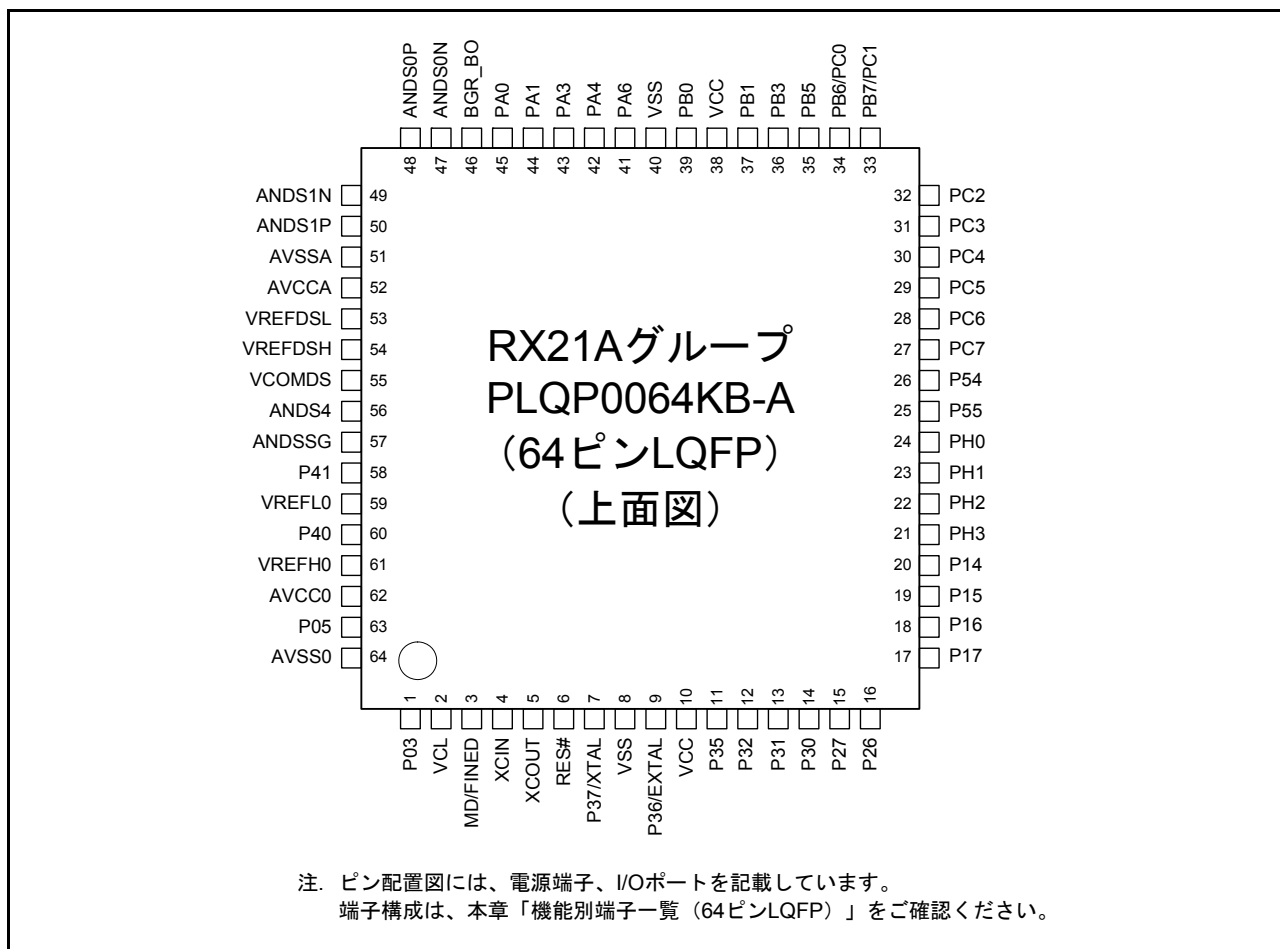
図 1.5 64 ピン LQFP ピン配置図
