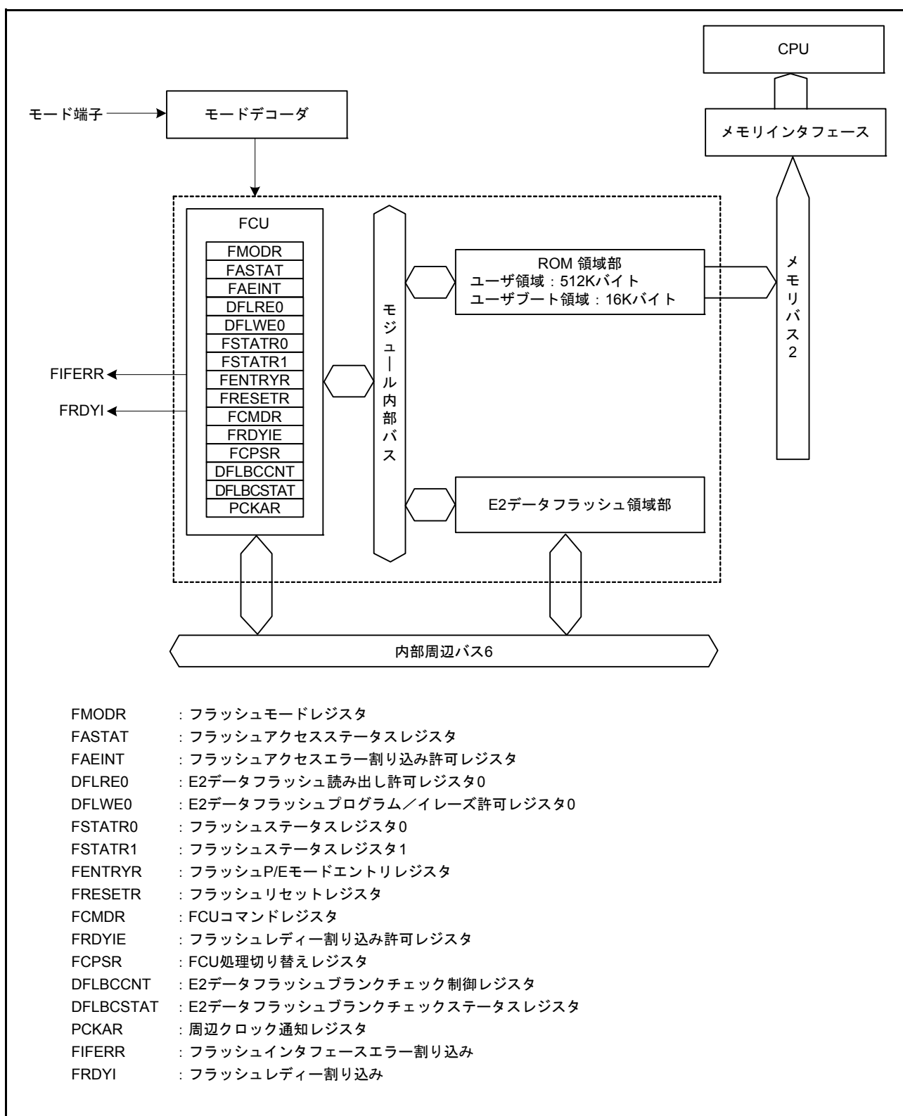
図 42.1 ROM のブロック図
