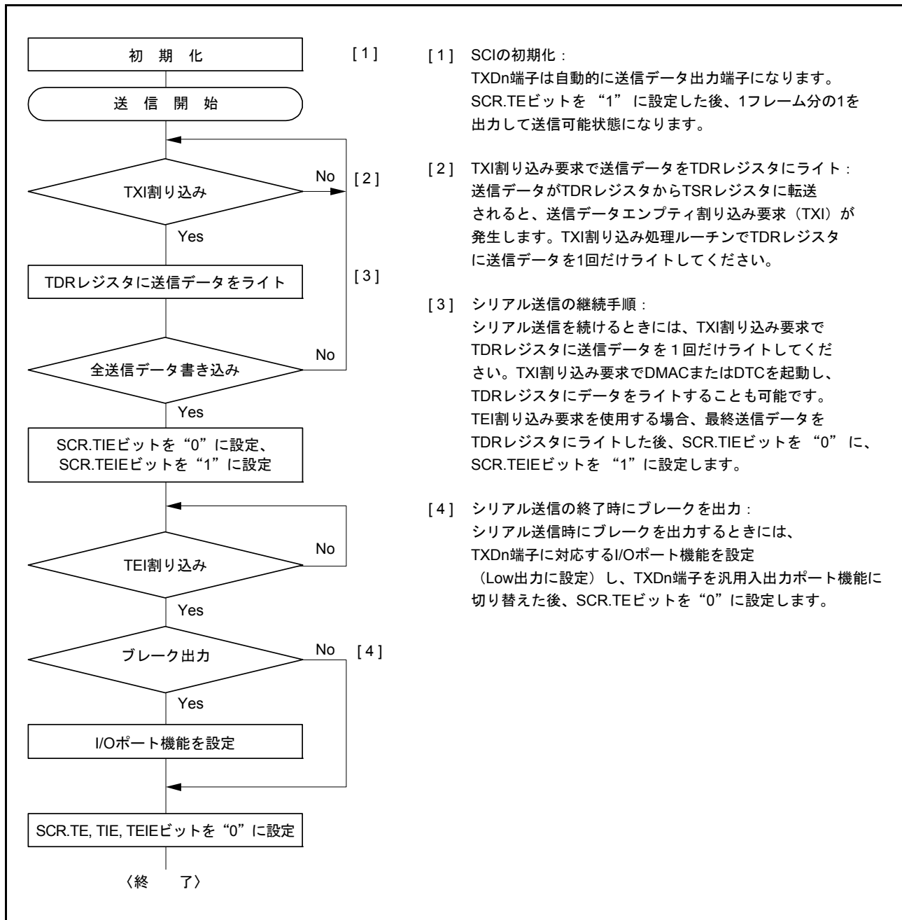
図 29.9 調歩同期式モードのシリアル送信のフローチャート例
