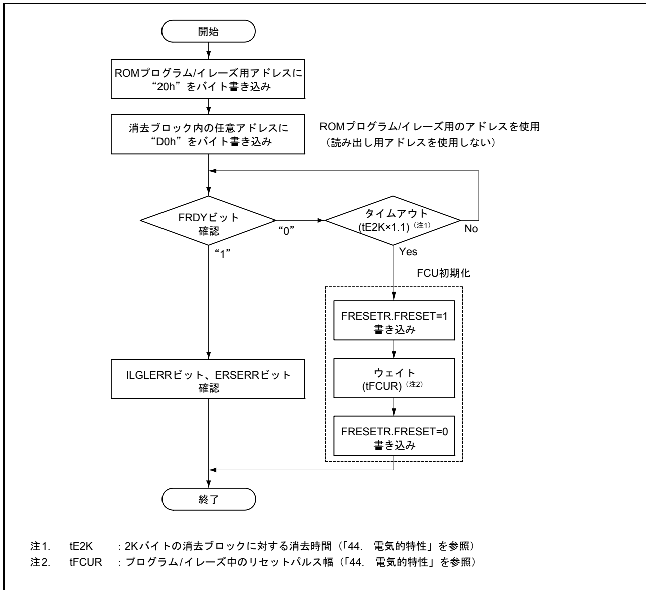
図 42.13 ROM イレーズ方法
