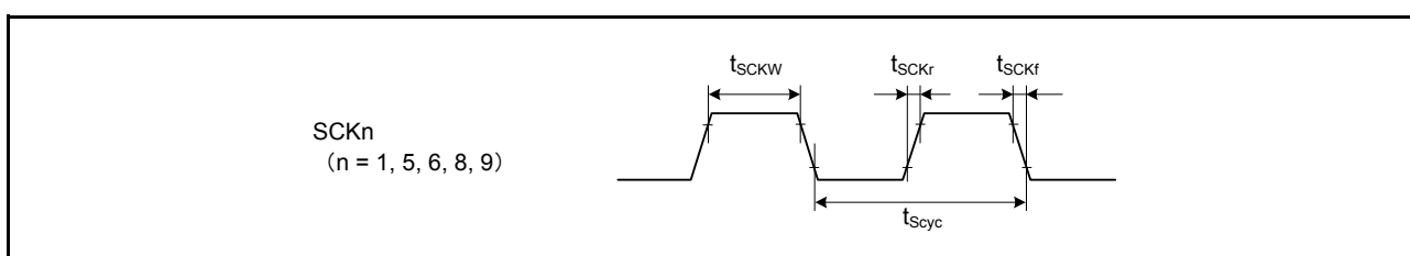
図 44.46 SCKクロック入力タイミング
