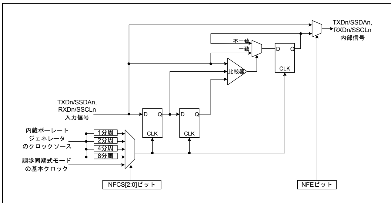
図 29.52 デジタルノイズフィルタ回路のブロック図
