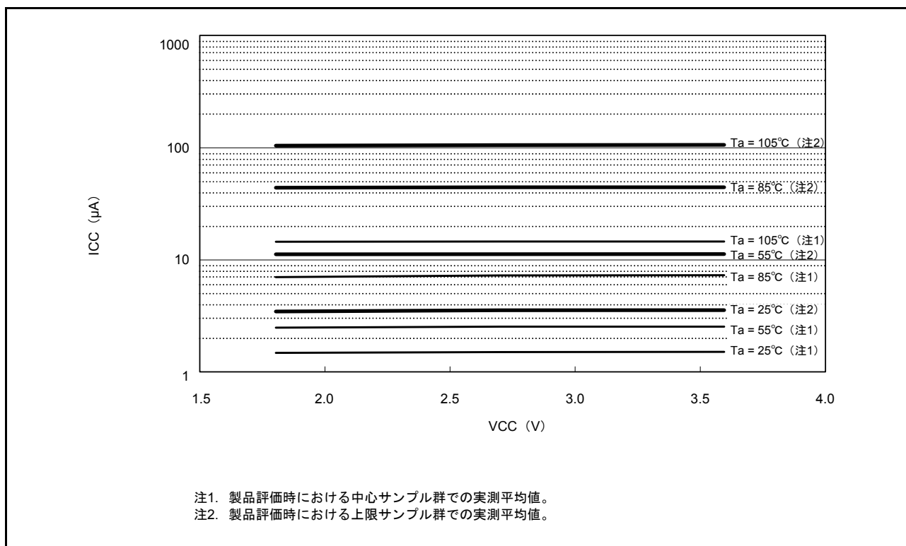
図 44.6 ソフトウェアスタンバイモード (SOFTCUT[2:0] ビット = 110b) 時の電圧依存性 (参考データ)
