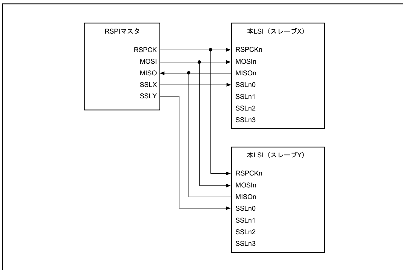
図 32.9 シングルマスタ / マルチスレーブの構成例 (本 LSI = スレーブ)
