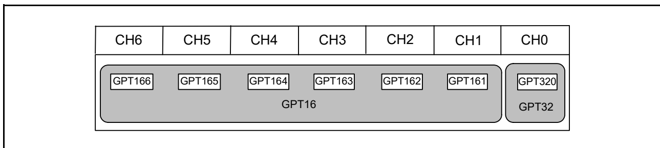
図 21.2 GPT の各チャンネルとモジュール名との対応
