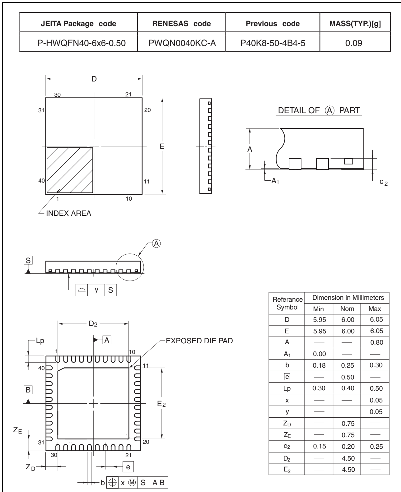
図 2.5 QFN 40 ピン
