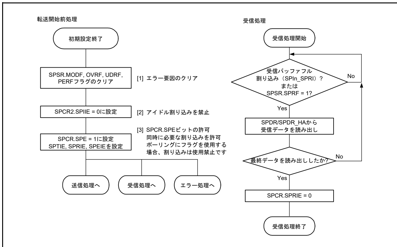
図 30.38 スレーブモード時の受信フロー
