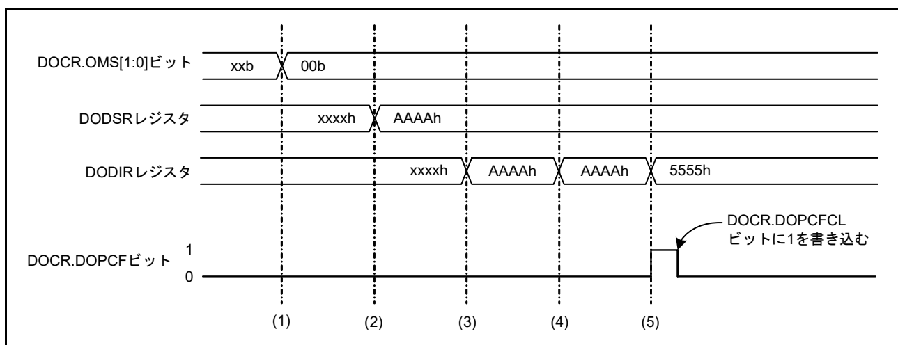
図 41.2 データ比較モードの動作例
