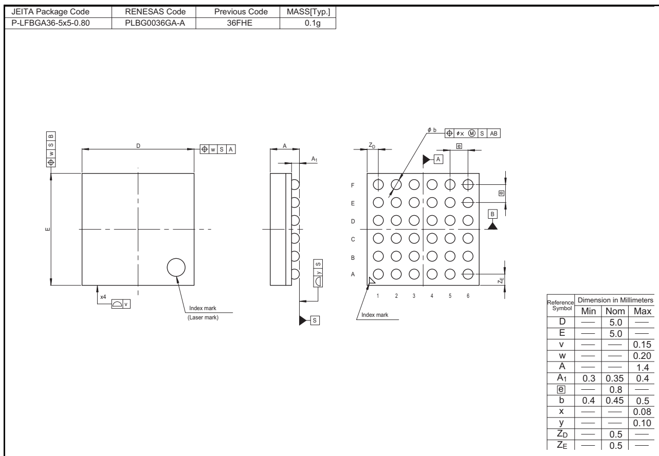
図 2.3 BGA 36 ピン
