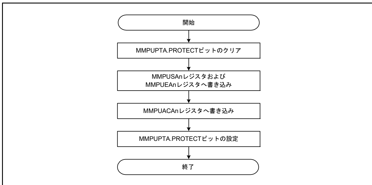
図 15.8 領域追加のレジスタ設定フロー
