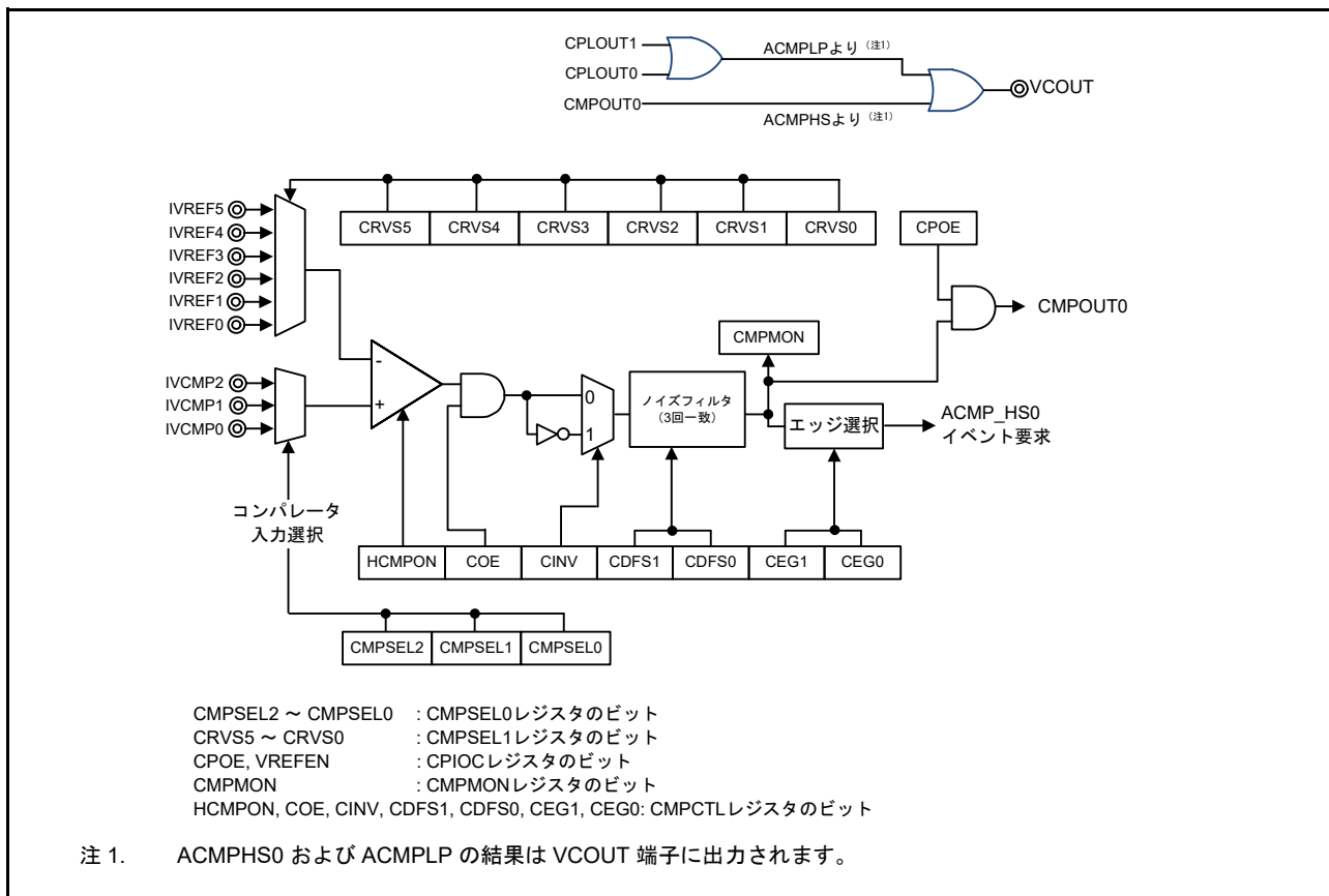
図 38.1 ACMPHS のブロック図
