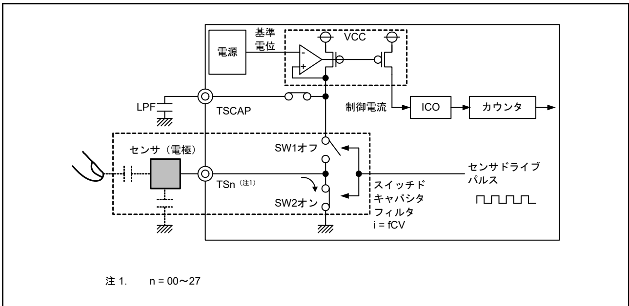
図 40.6 放電動作
