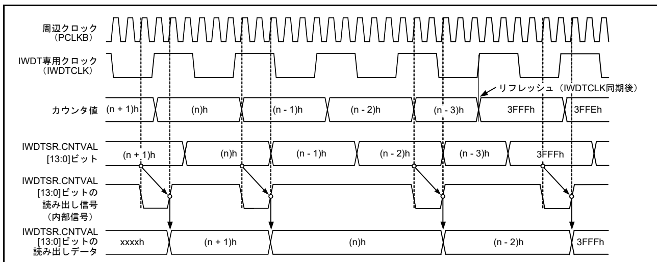
図 25.5 IWDT カウンタ値の読み出し処理 (OFS0.IWDTCK3[3:0] = 0000b、OFS0.IWDTTOPS[1:0] = 11b の場合)
