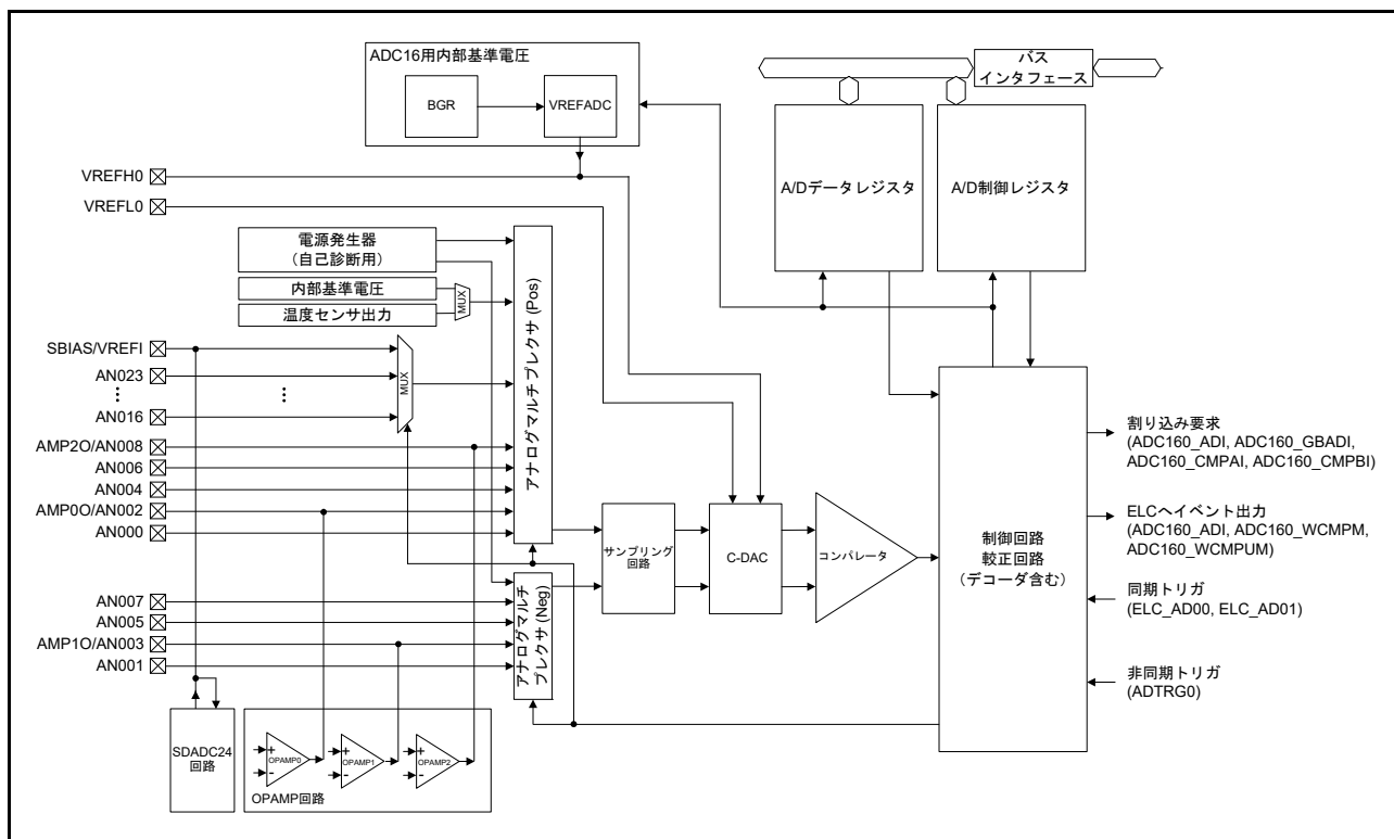
図 32.1 ADC16のブロック図
