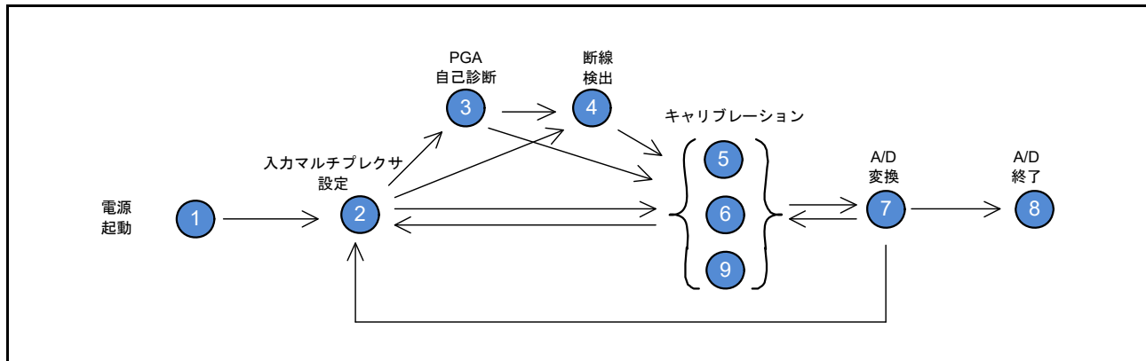
図 33.22 フロー概要
