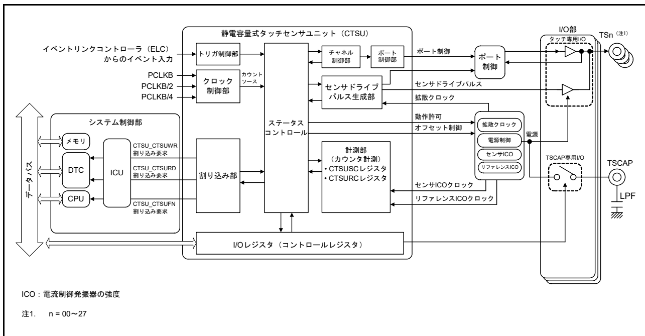
図 40.3 CTSUS のブロック図
