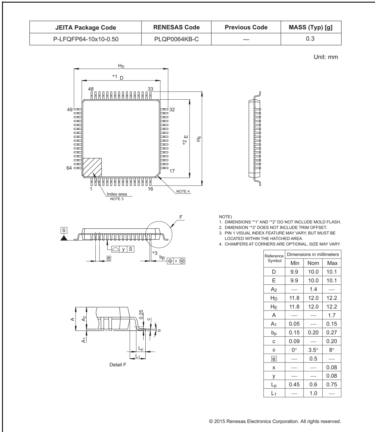
図 2.1 LQFP 64 ピン
