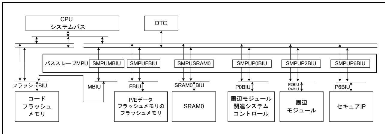
図 15.9 バススレーブ MPU のブロック図
