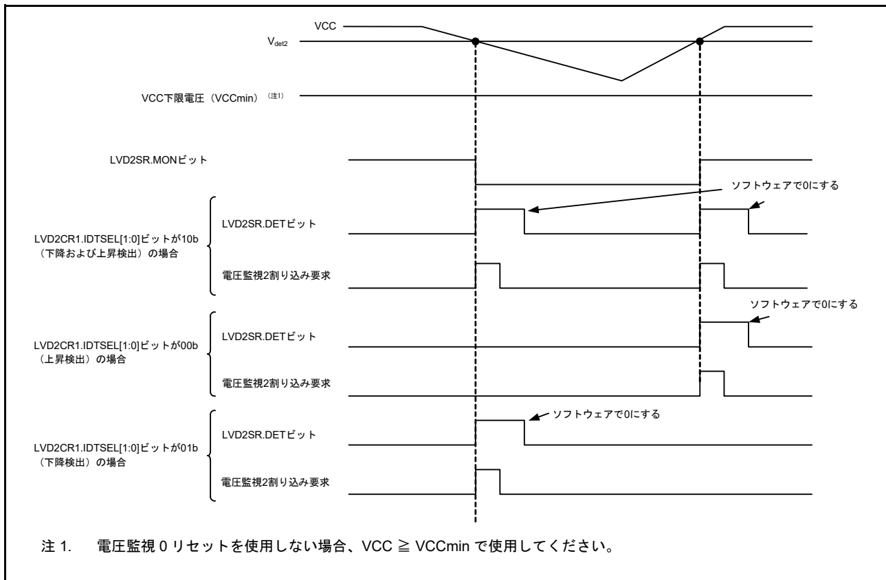
図 8.6 電圧監視 2 割り込みの動作例
