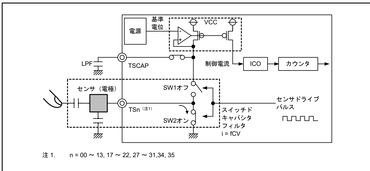
図 41.6 放電動作
