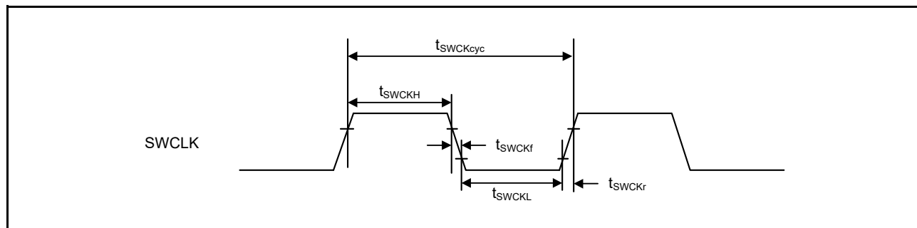
図 47.86 SWD SWCLK タイミング
