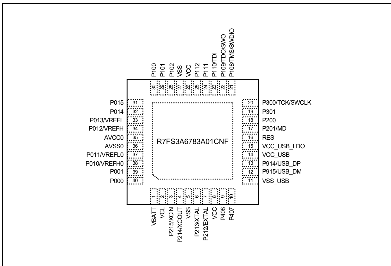
図 1.9 40-pin QFN のピン配置図 (上面図)
