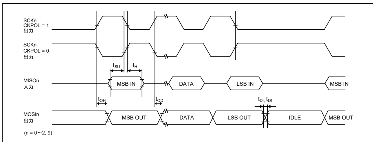
図 47.48 SCI 簡易 SPI モードタイミング (マスタ、CKPH = 0)
