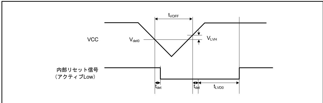
図 47.74 電圧検出回路タイミング ( V_{det0} )
