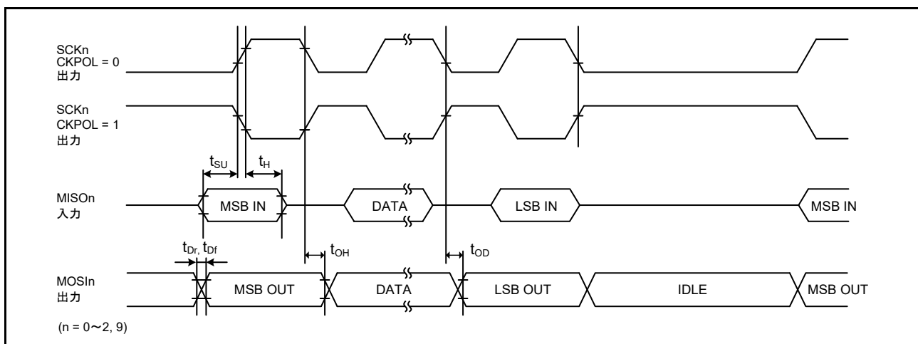
図 47.47 SCI 簡易 SPI モードタイミング (マスタ、CKPH = 1)
