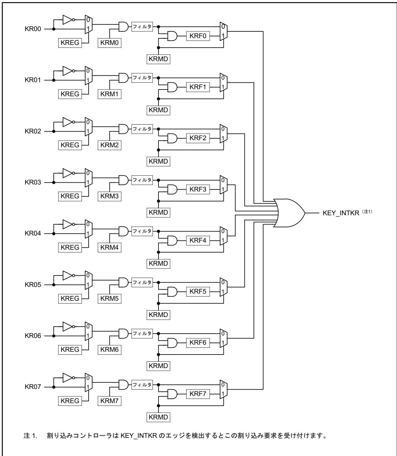
図 20.1 キー割り込み機能のブロック図
