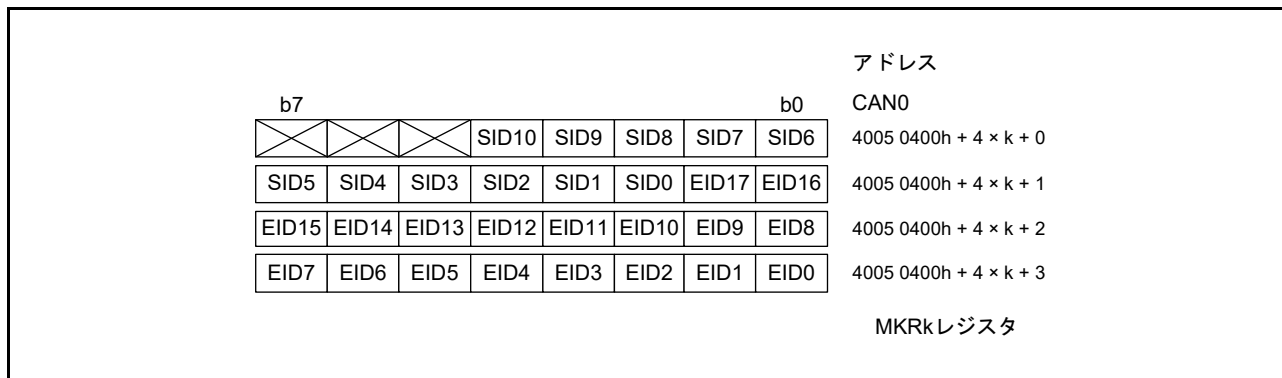
図 30.14 MKRk レジスタの構成 (k = 0 ~ 7)
