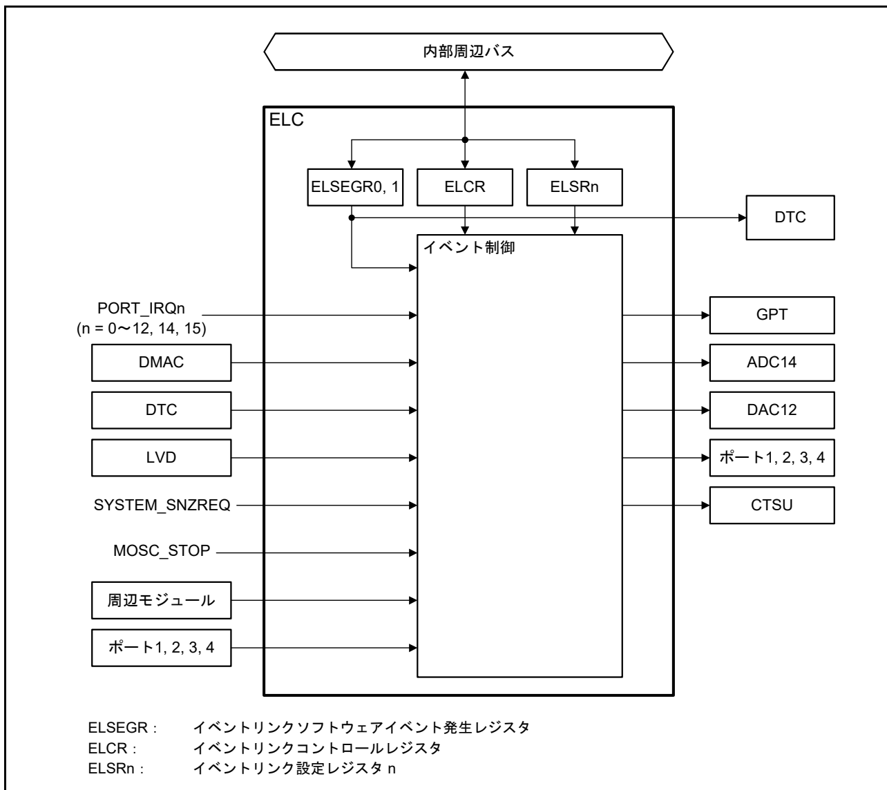
図 18.1 ELC のブロック図 (n = 0 ~ 9, 12, 14 ~ 18)
