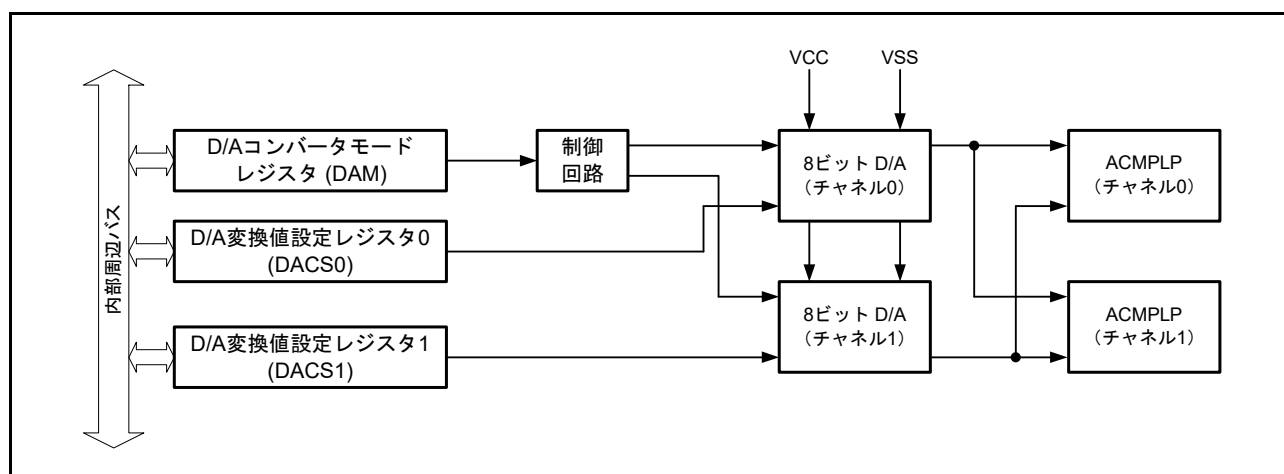
図 40.1 8ビットD/Aコンバータのブロック図
