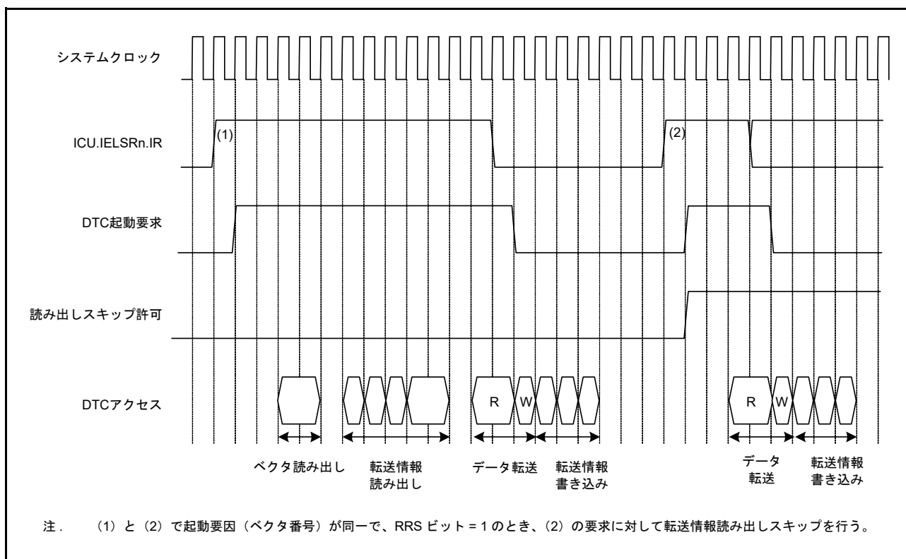
図 17.12 転送情報の読み取りスキップ時の動作例 (ベクタ、転送情報、転送先データが SRAM にあり、転送元データが周辺モジュールにある場合)
