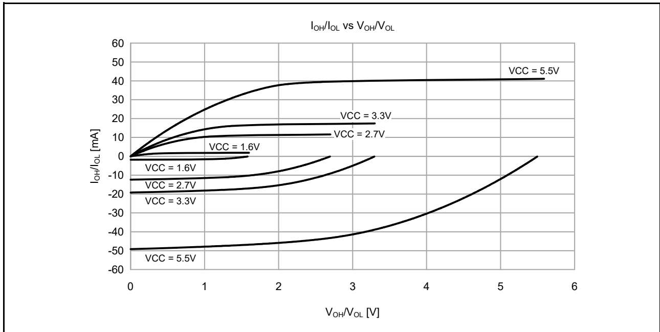
図 47.2 低駆動出力選択時の T_a = 25^\circ\text{C} での V_{OH}/V_{OL} および I_{OH}/I_{OL} 電圧特性 (参考データ)
