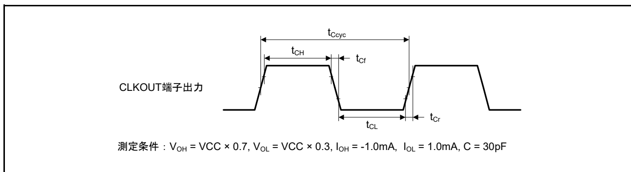
図 47.64 CLKOUT 出力タイミング
