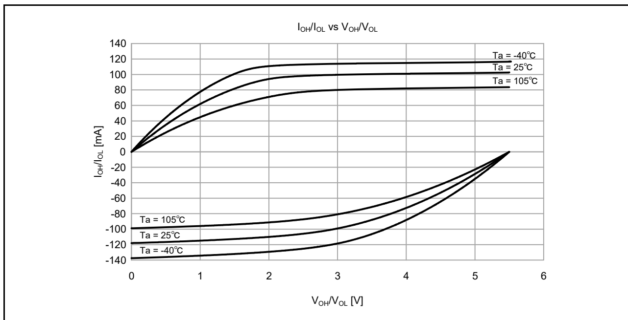
図 47.11 中駆動出力選択時の V_{CC} = 5.5V での V_{OH}/V_{OL} および I_{OH}/I_{OL} 温度特性 (参考データ)
