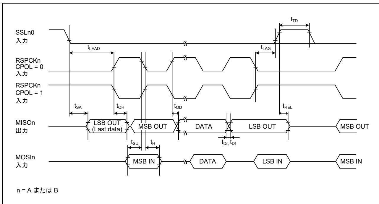
図 47.58 SPI タイミング (スレーブ、CPHA = 1)
