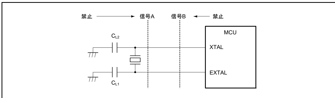
図 8.8 発振回路部のボード設計での信号ルーティング (メインクロック発振器の場合、サブクロック発振器も同様)
