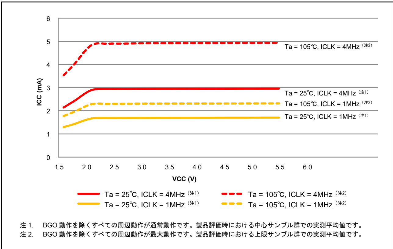
図 47.20 Low-voltage モードにおける電圧依存性 (参考データ)
