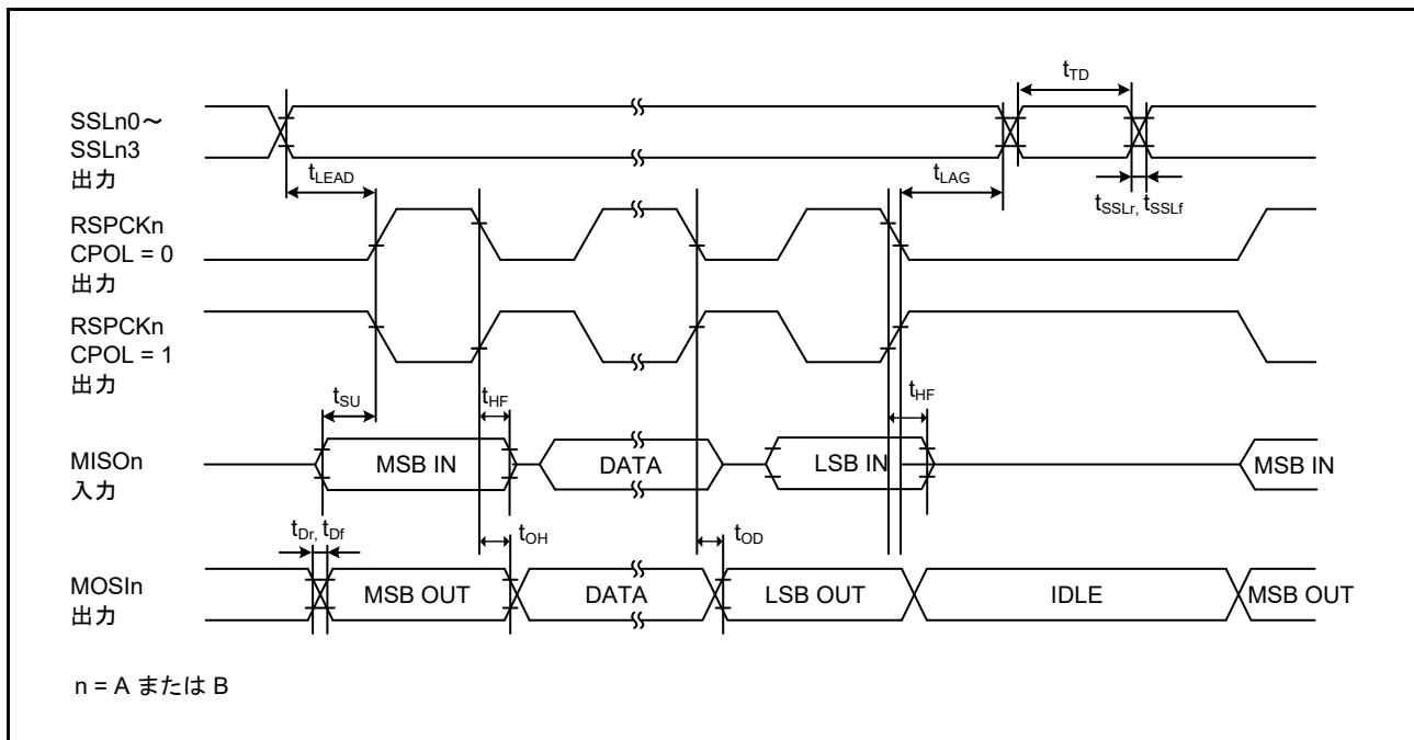
図 47.54 SPI タイミング (マスタ、CPHA = 0) (ビットレート : PCLKA を 2 分周に設定)
