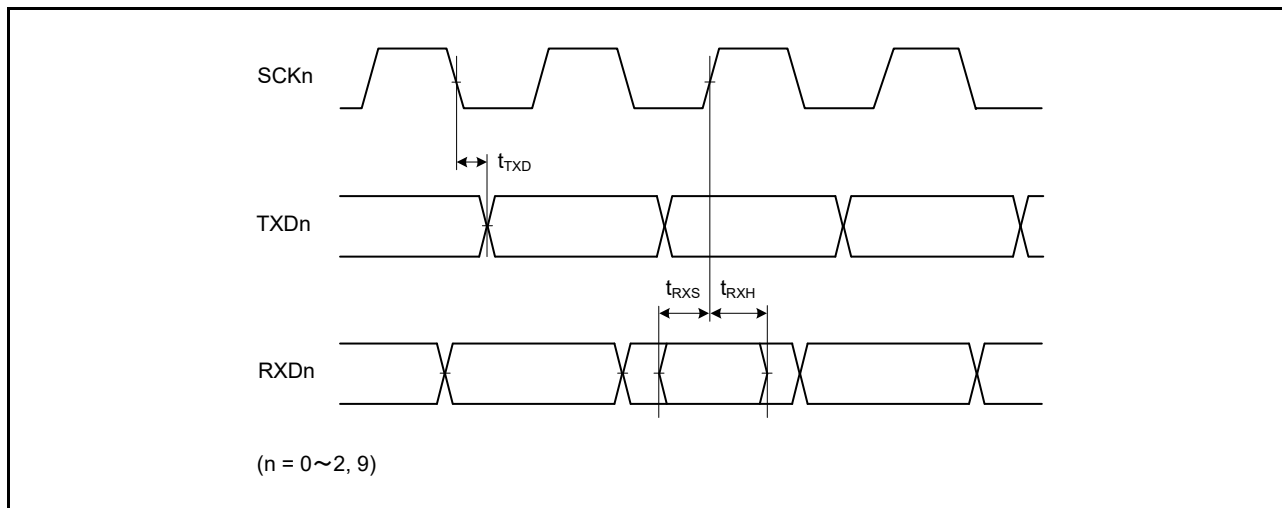
図 47.45 クロック同期式モードにおける SCI 入出力タイミング
