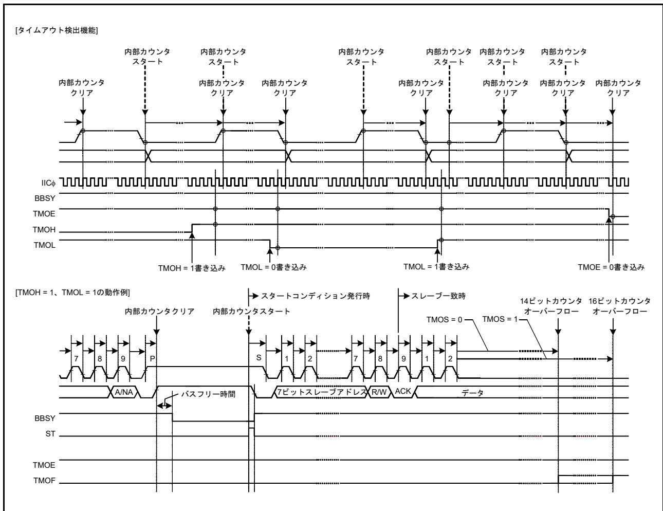
図 29.48 タイムアウト検出機能 (TMOE、TMOS、TMOH、TMOL ビット)
