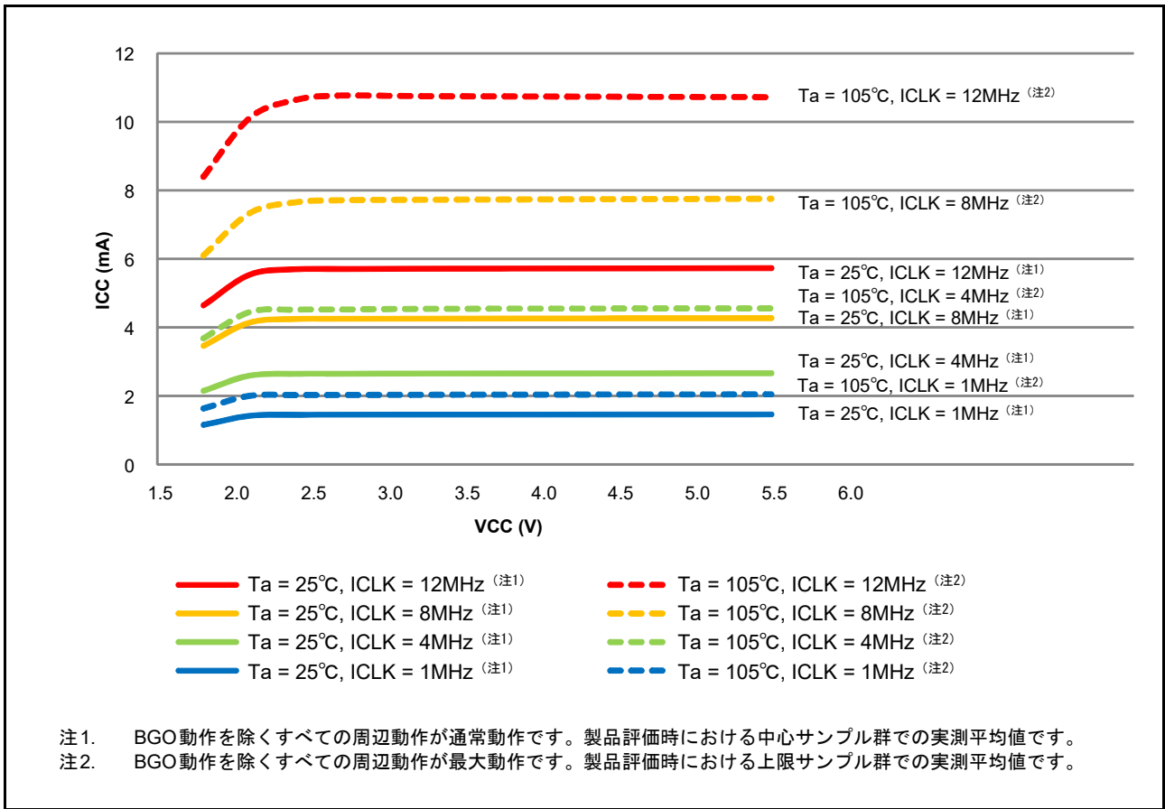
図 47.18 Middle-speed 動作モードにおける電圧依存性 (参考データ)
