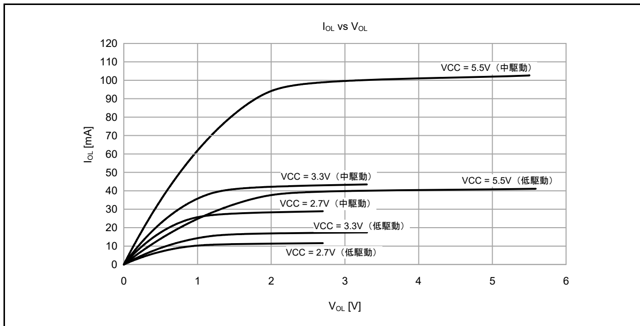
図 47.16 T_a = 25^\circ C での V_{OH}/V_{OL} および I_{OH}/I_{OL} 電圧特性
