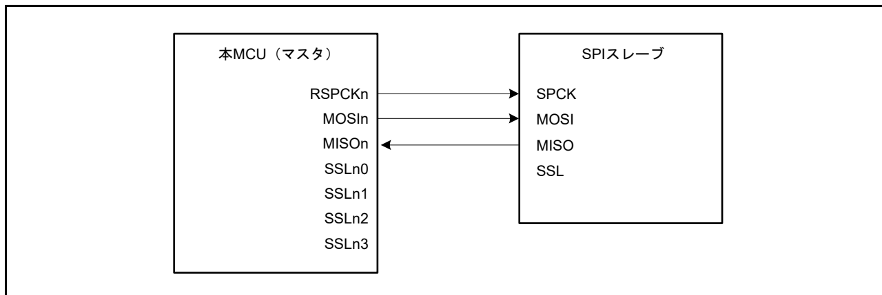
図 31.11 クロック同期モードのマスター/スレーブの構成例 (MCU はマスター)
