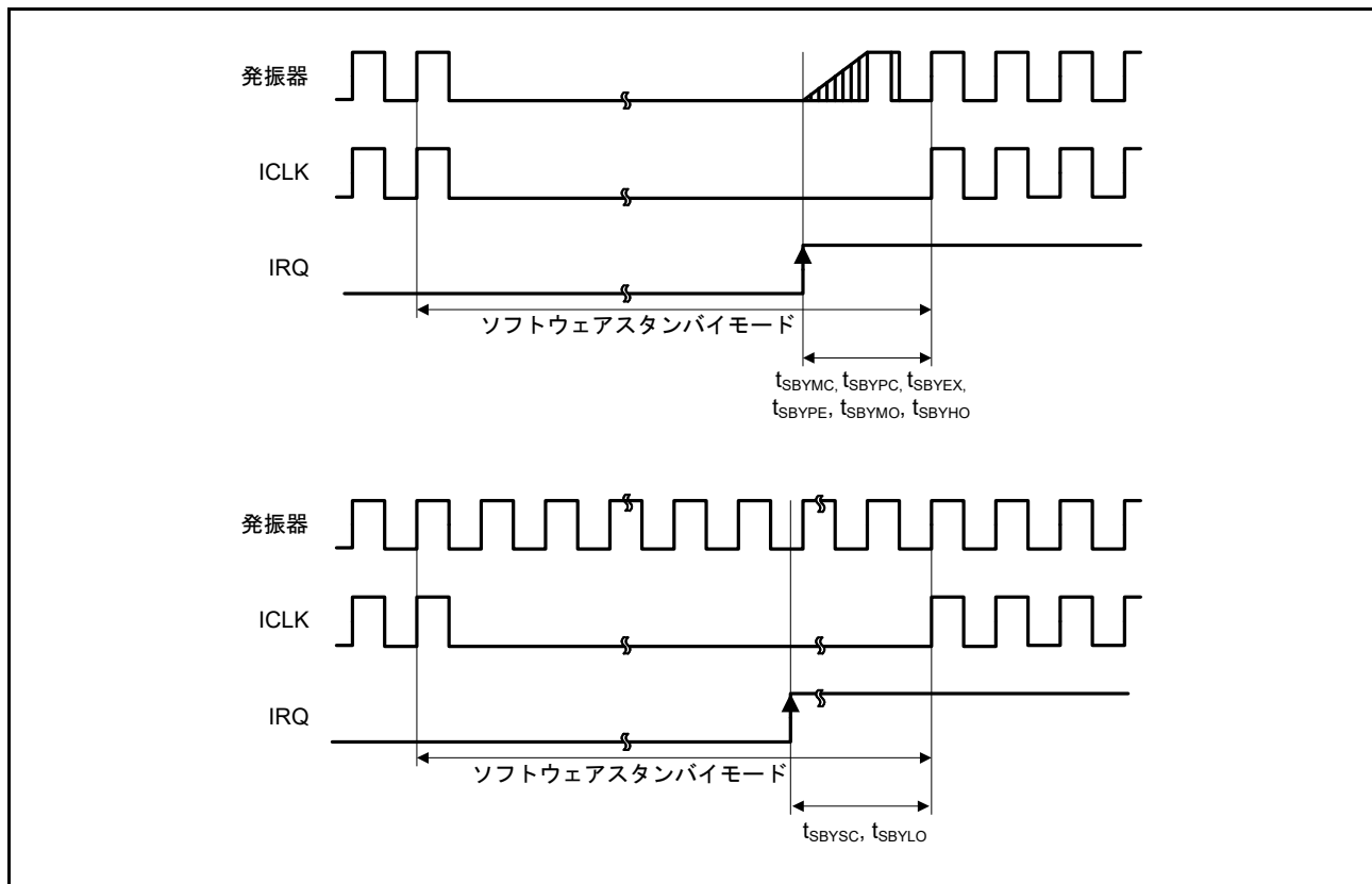
図 47.34 ソフトウェアスタンバイモード解除タイミング
