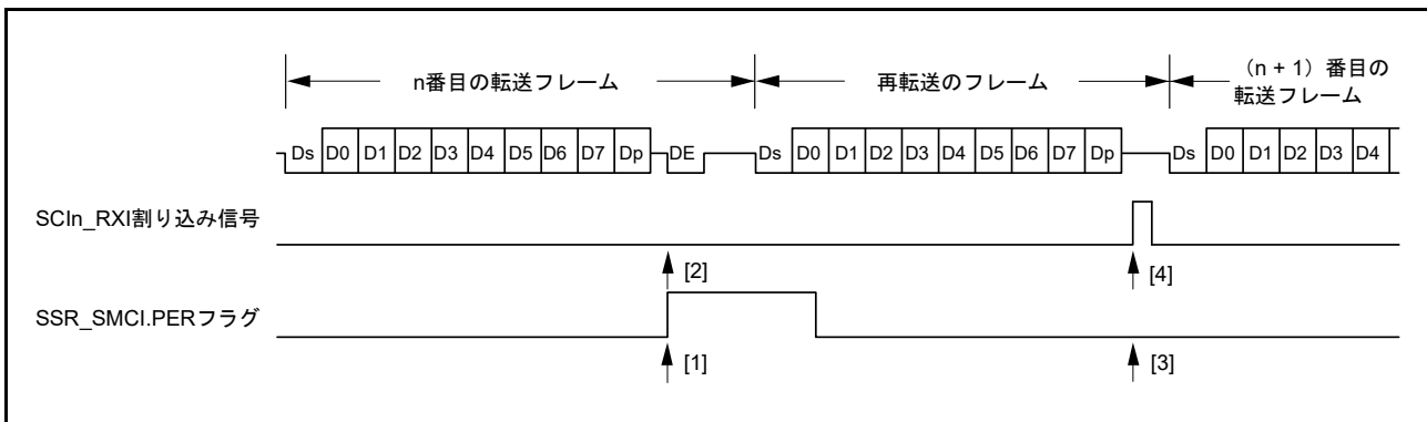
図 28.55 SCI 受信モードでの再転送動作（受信時の再転送動作）
