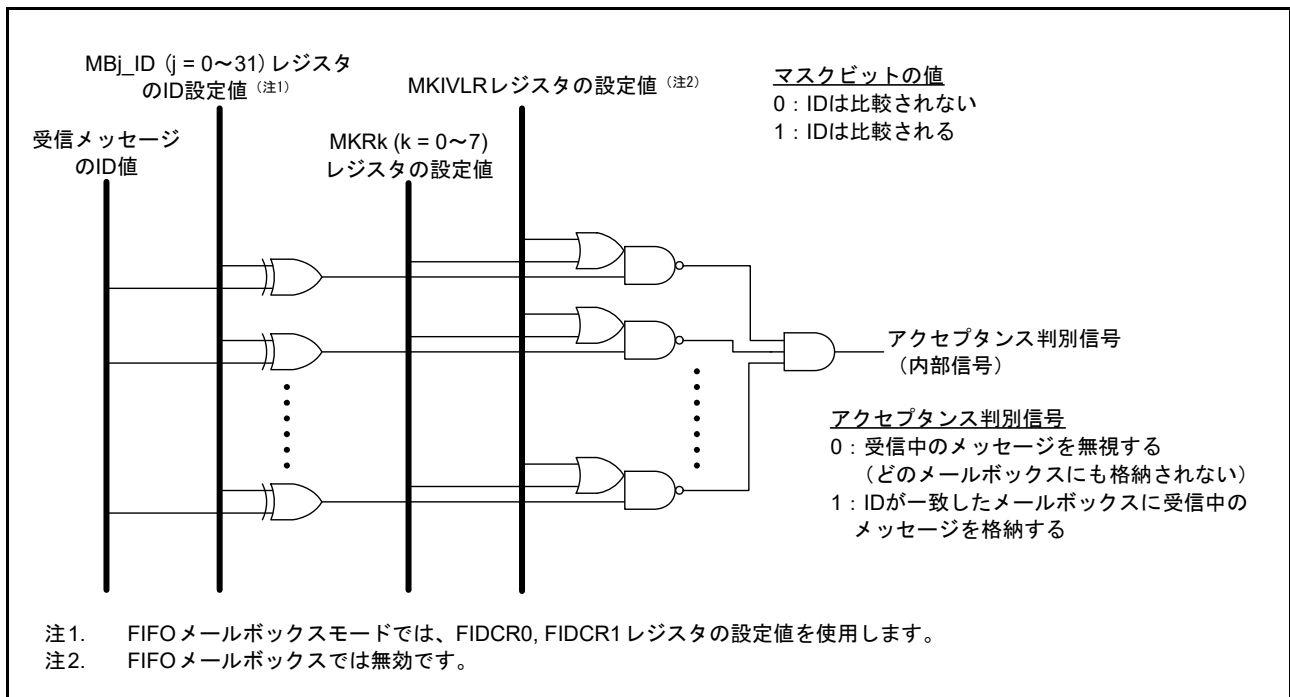
図 30.17 アクセプタンスフィルタ機能
