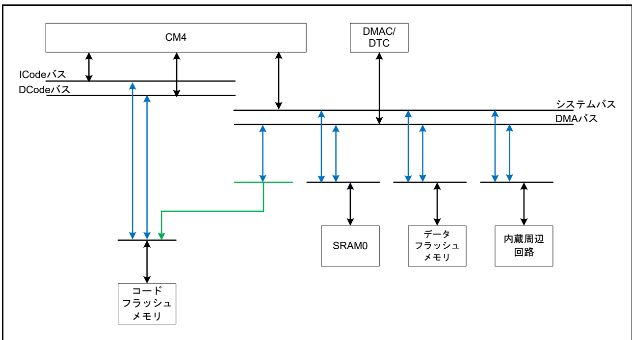
図 14.1 バスの構成図
