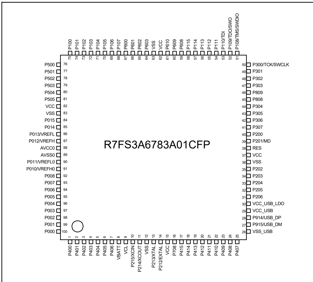
図 1.3 100-pin LQFP のピン配置図 (上面図)
