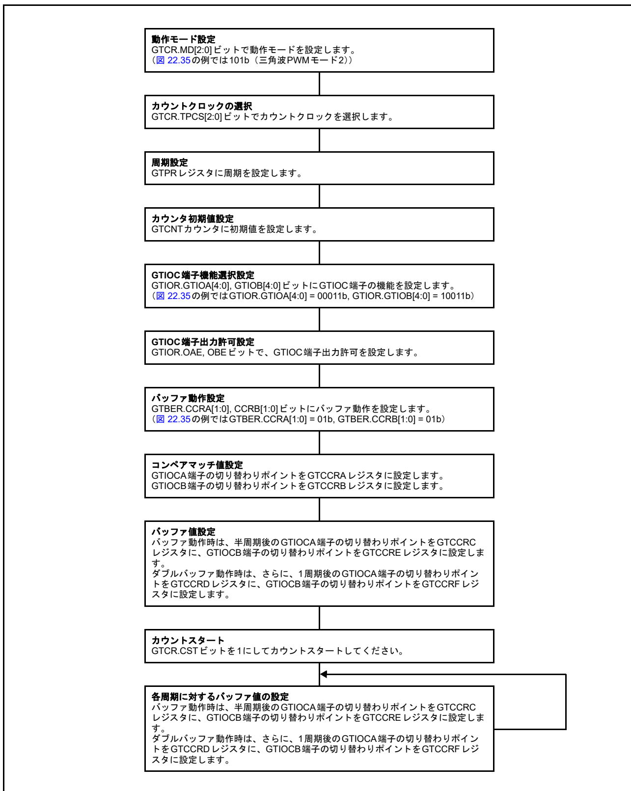
図 22.36 三角波 PWM モード 2 の設定例
