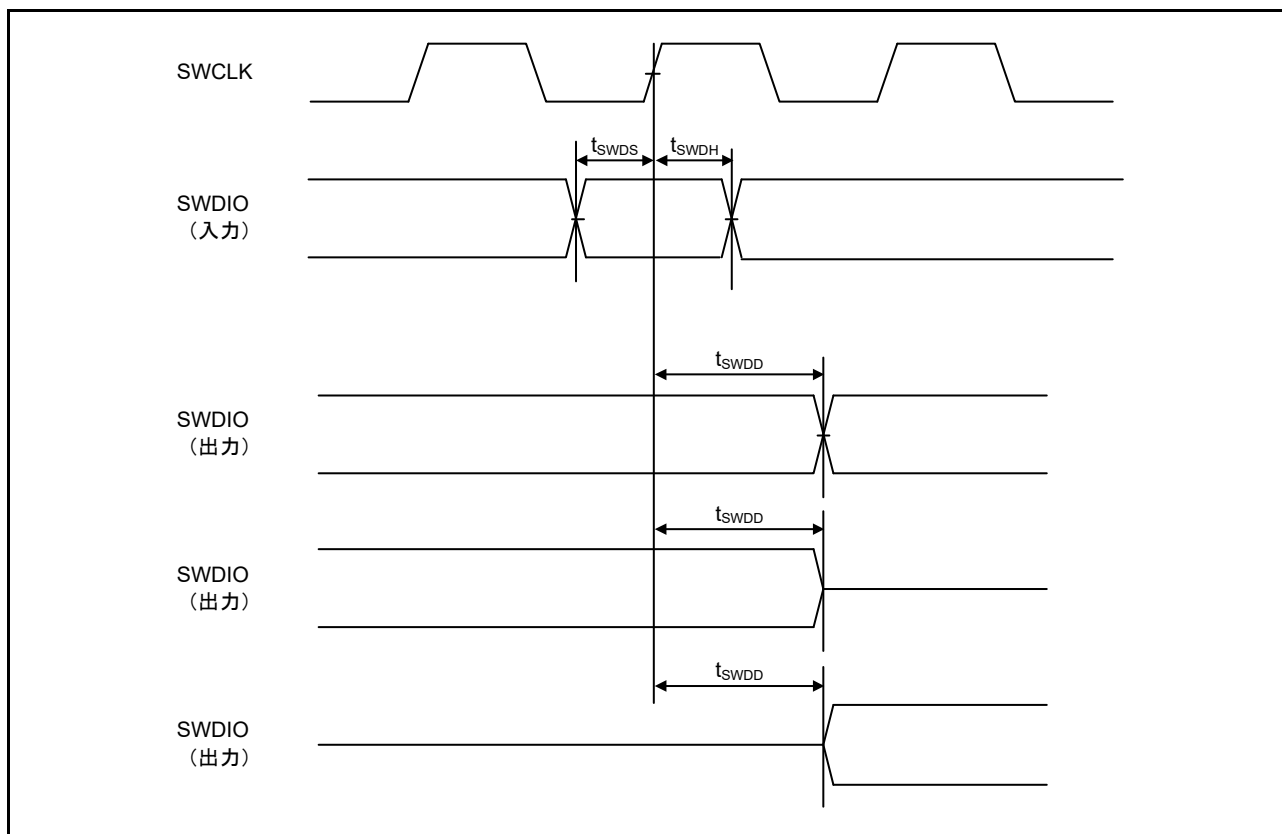
図 47.87 SWD 入出力タイミング
