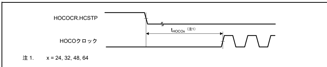
図 47.27 HOCO クロック発振開始タイミング (HOCOCCR.HCSTP ビット設定による開始)
