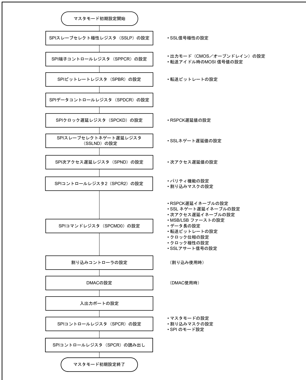
図 31.35 マスタモード時の SPI 動作の初期化フロー例
