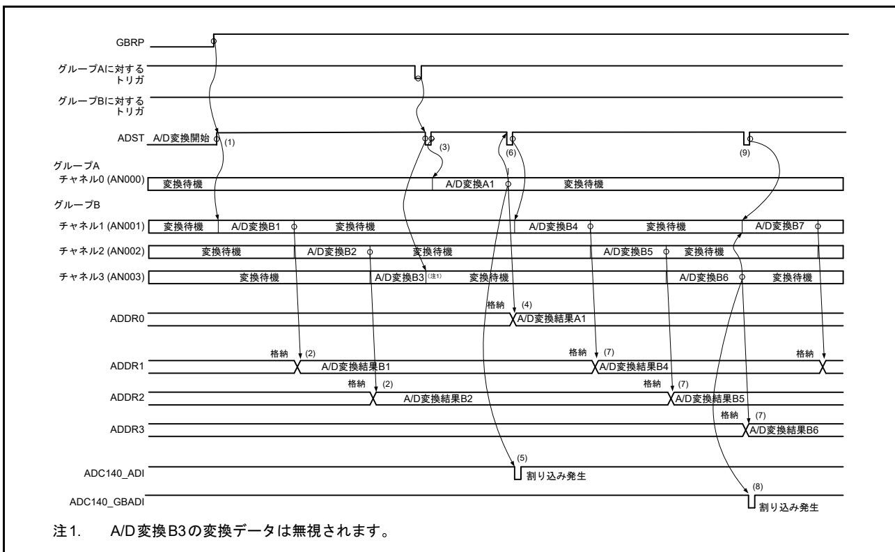
図 35.20 グループ A 優先制御の動作例 (5) (ADGSPCR.GBRP = 1 の場合)
