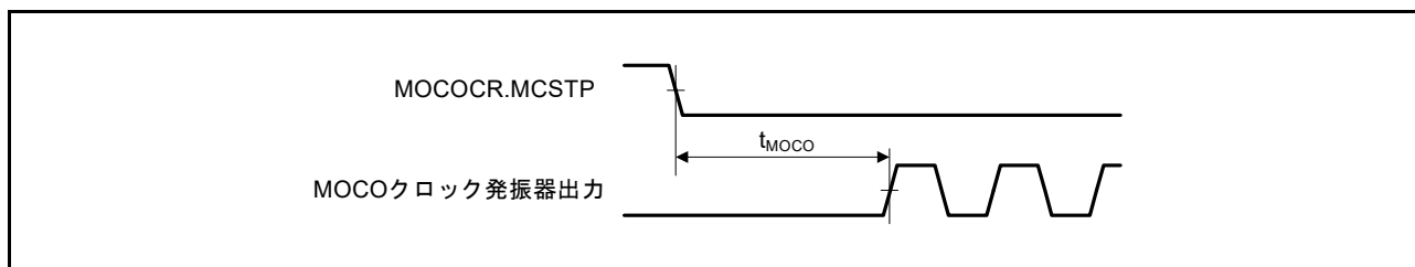
図 47.31 MOCO クロック発振開始タイミング
