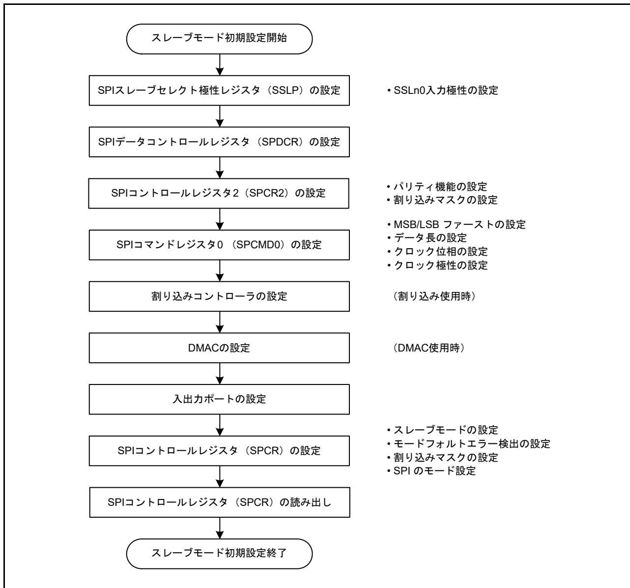
図 31.39 スレーブモード時の SPI 動作の初期化フロー例
