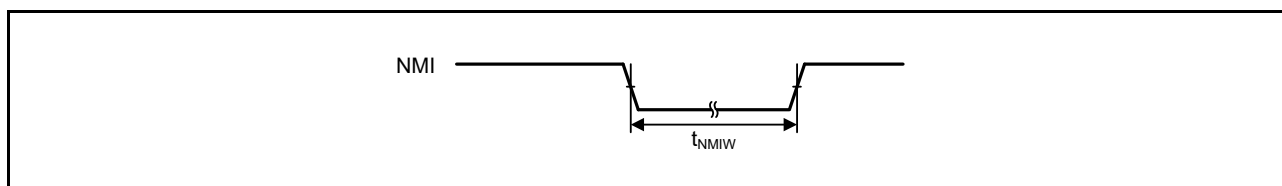
図 47.36 NMI 割り込み入力タイミング
