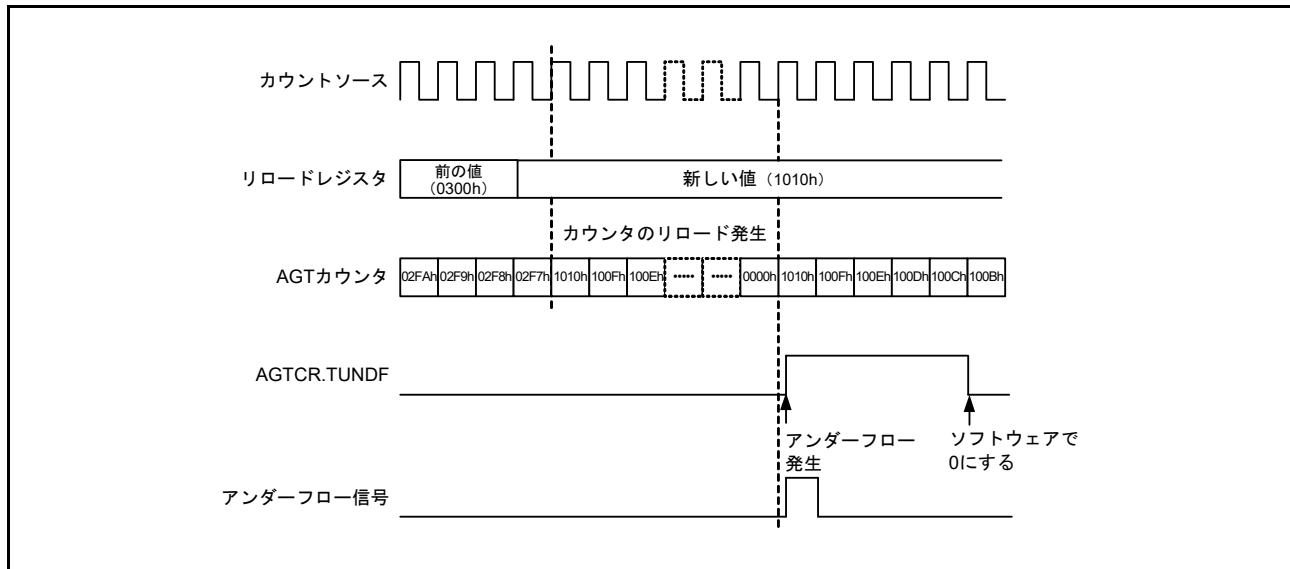
図 23.5 タイマモードでの動作例
