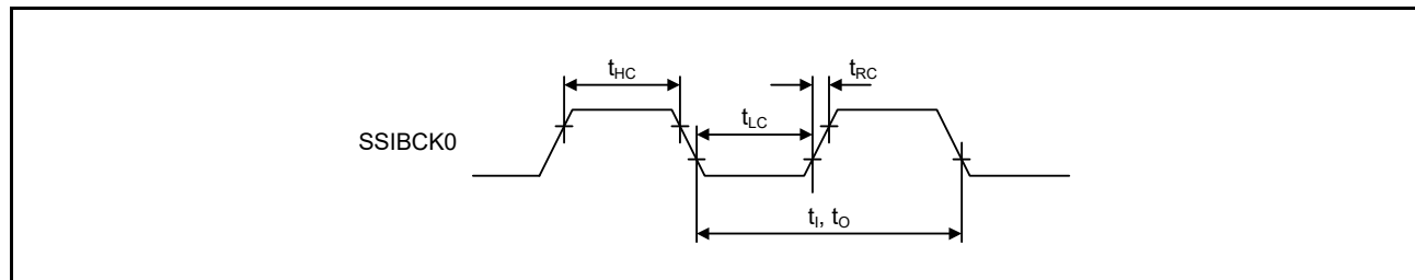
図 47.60 SSIE クロック入出力タイミング
