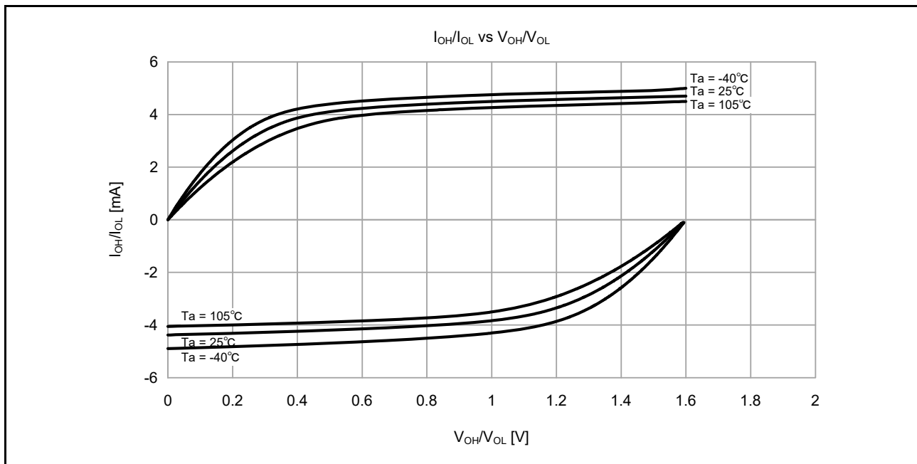
図 47.8 中駆動出力選択時の VCC = 1.6V での V OH /V OL および I OH /I OL 温度特性 (参考データ)
