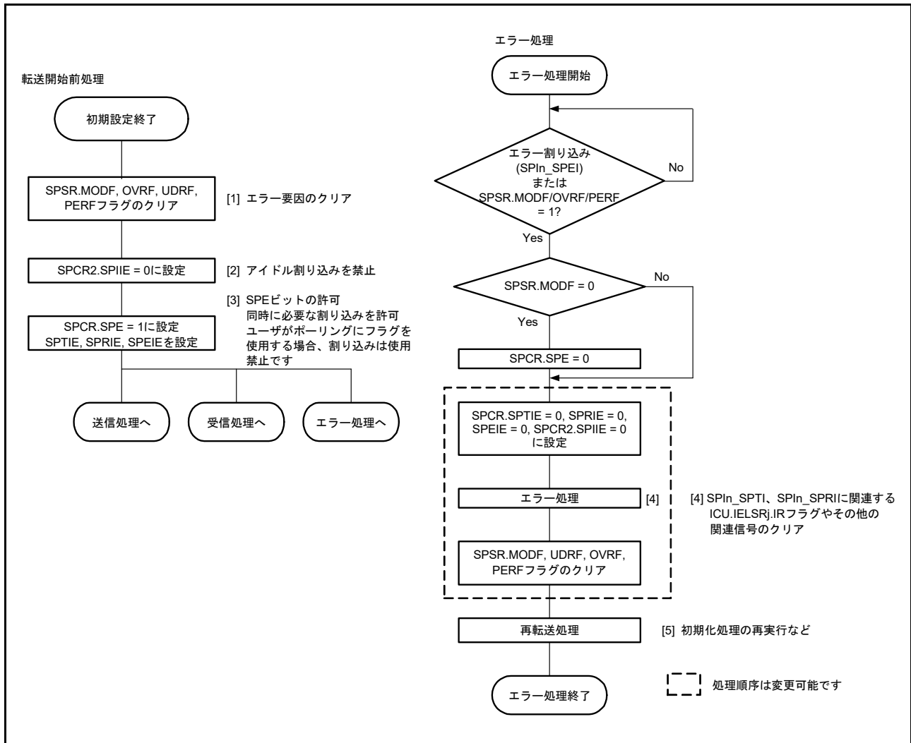
図 31.42 スレーブモードでのエラー処理フロー
