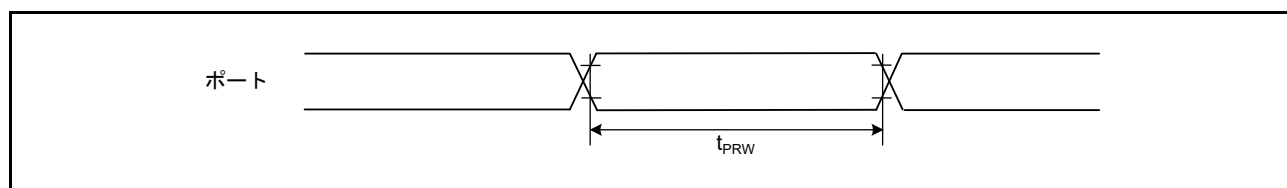
図 47.38 I/Oポート入力タイミング
