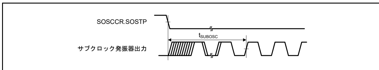
図 47.30 サブクロック発振開始タイミング
