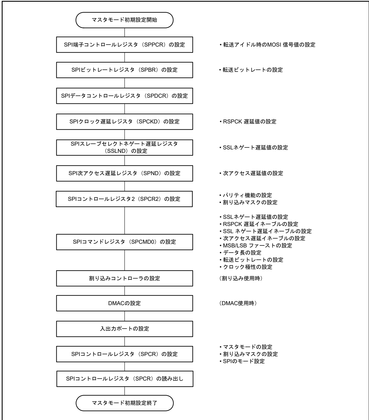
図 31.46 マスタモード時のクロック同期式動作の初期化フロー例
