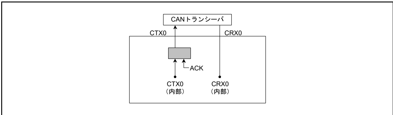
図 30.7 セルフテストモード 0 選択時の接続
