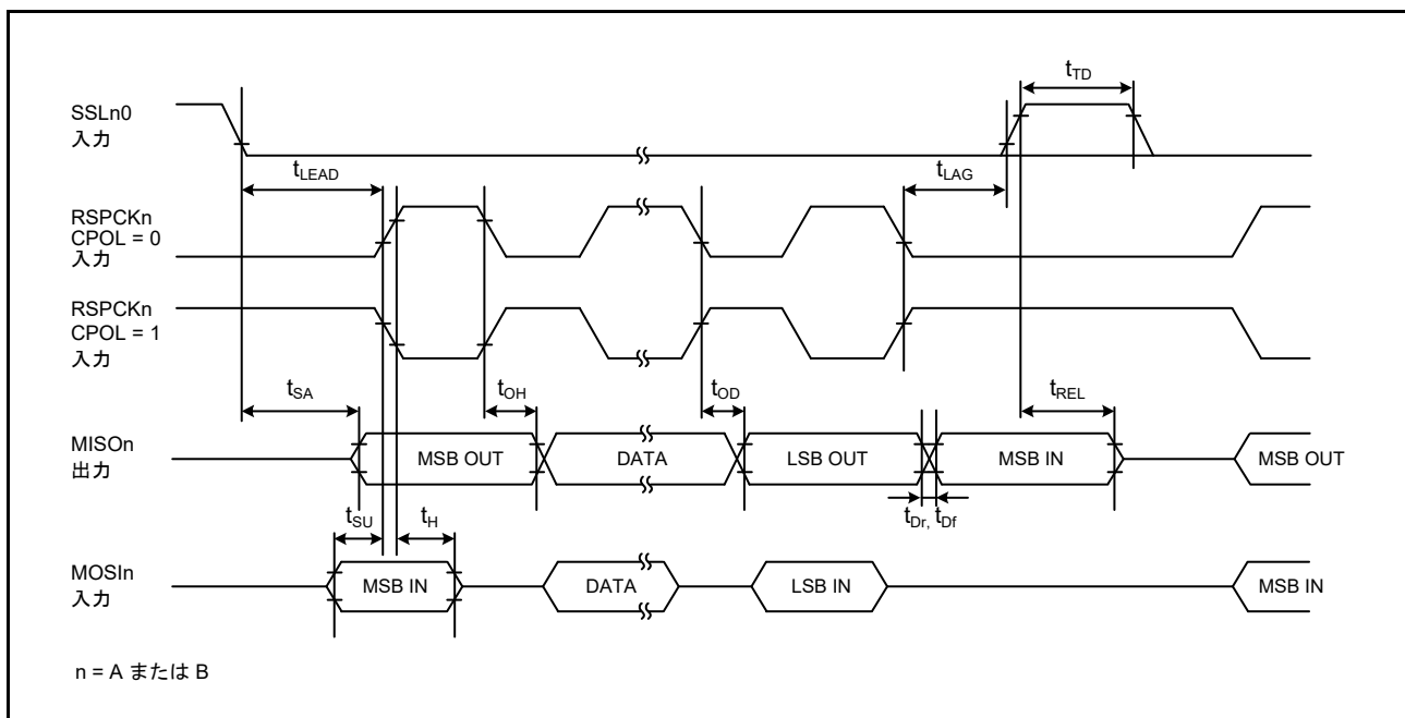
図 47.57 SPI タイミング (スレーブ、CPHA = 0)
