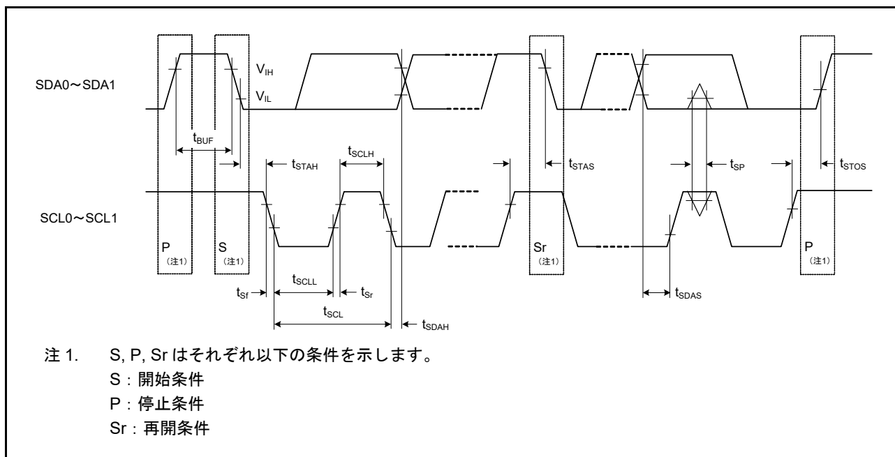
図 47.59 I2C バスインタフェース入出タイミング
