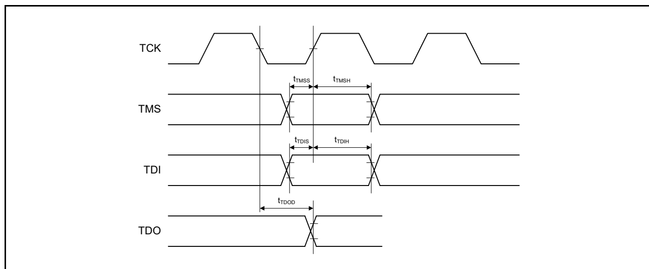
図 47.82 バウンダリスキャン入出力タイミング
