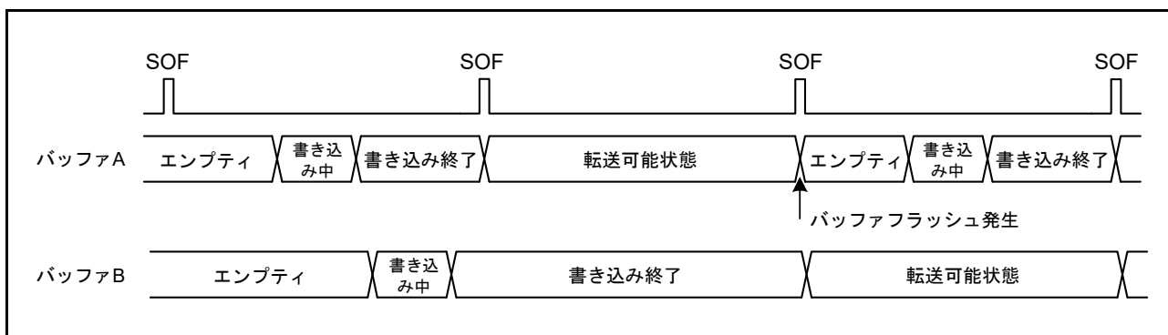
図 27.22 バッファフラッシュ動作例
