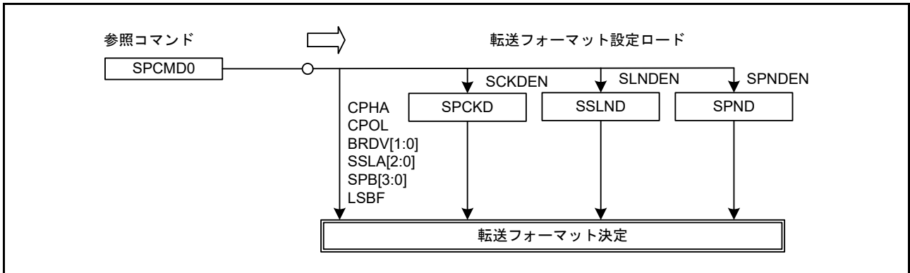
図 31.43 マスタモードでのシリアル転送フォーマットの決定方法
