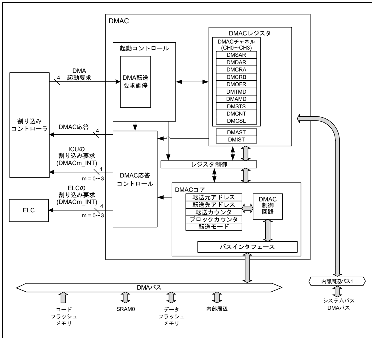
図 16.1 DMAC のブロック図
