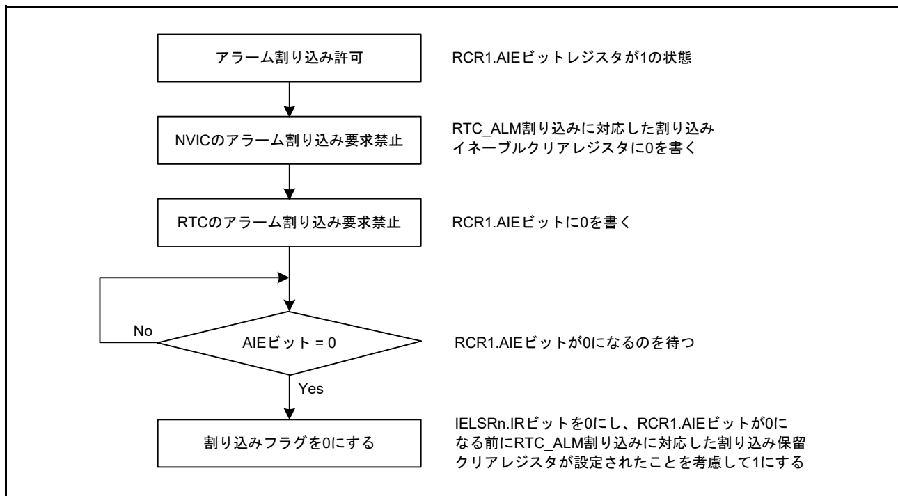
図 24.8 アラーム割り込み要求の禁止手順
