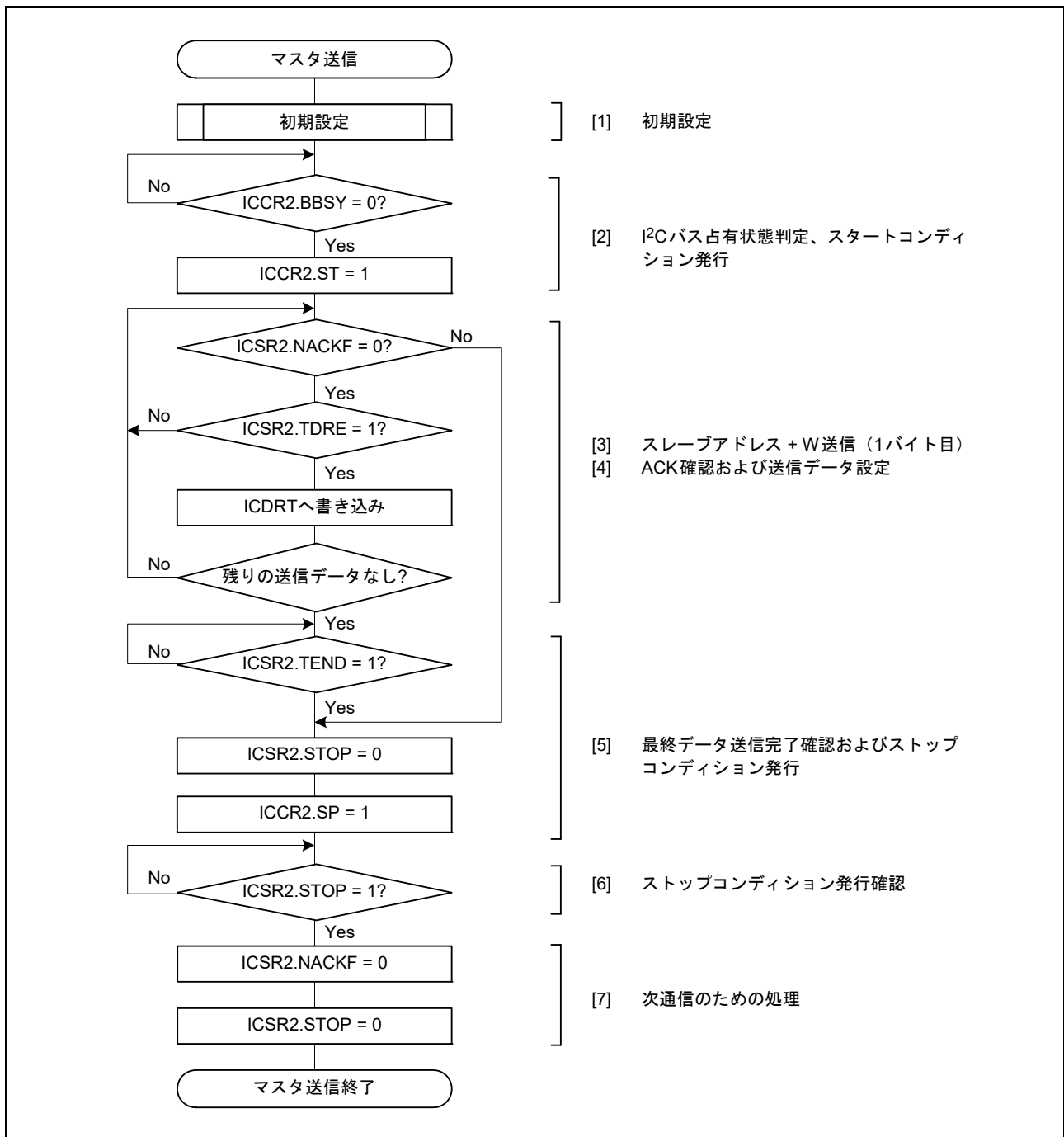
図 29.6 マスタ送信のフローチャート例
