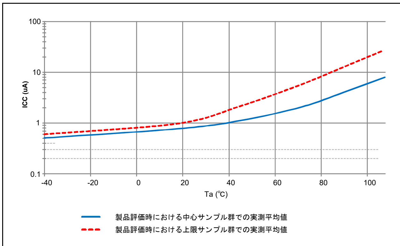
図 47.22 すべての SRAM がオンのソフトウェアスタンバイモード時の温度依存性 (参考データ)
