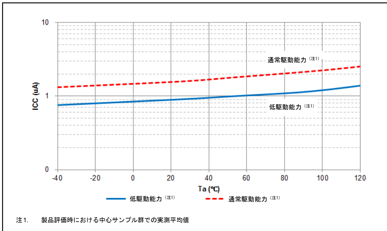
図 47.23 VCC オフ時の RTC 動作の温度依存性 (参考データ)
