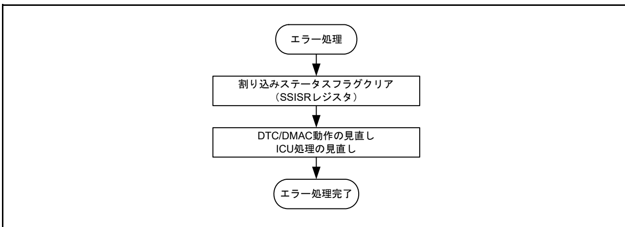
図 33.53 エラー処理手順
