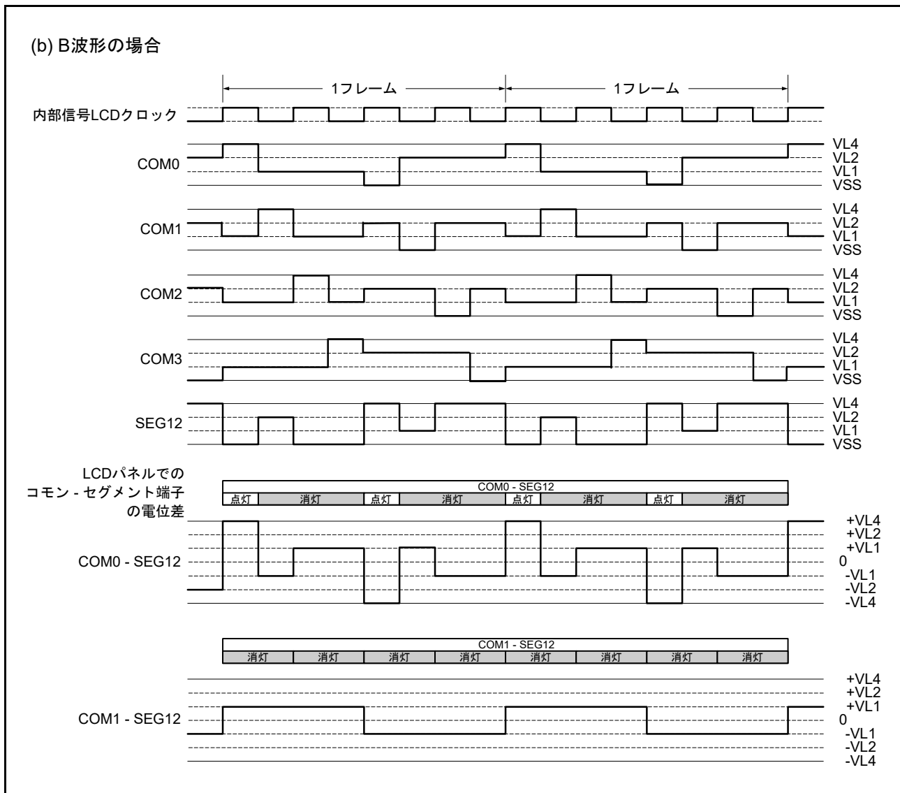
図 45.31 1/3 バイアス法を用いた SEG12 と各コモン信号との間の 4 時分割 LCD 駆動波形例 (2/2)
