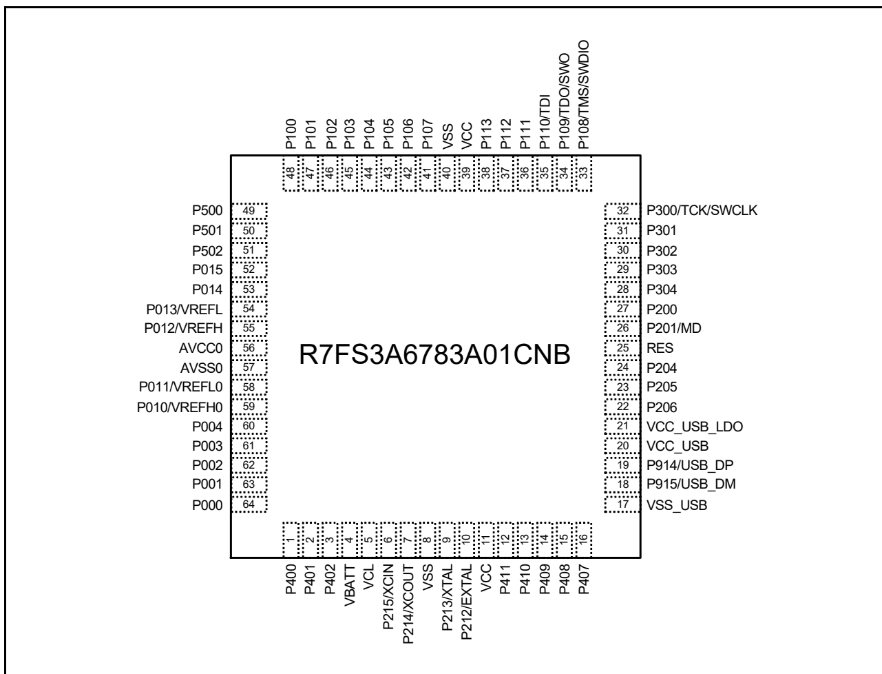
図 1.6 64-pin QFN のピン配置図 (上面透視図)
