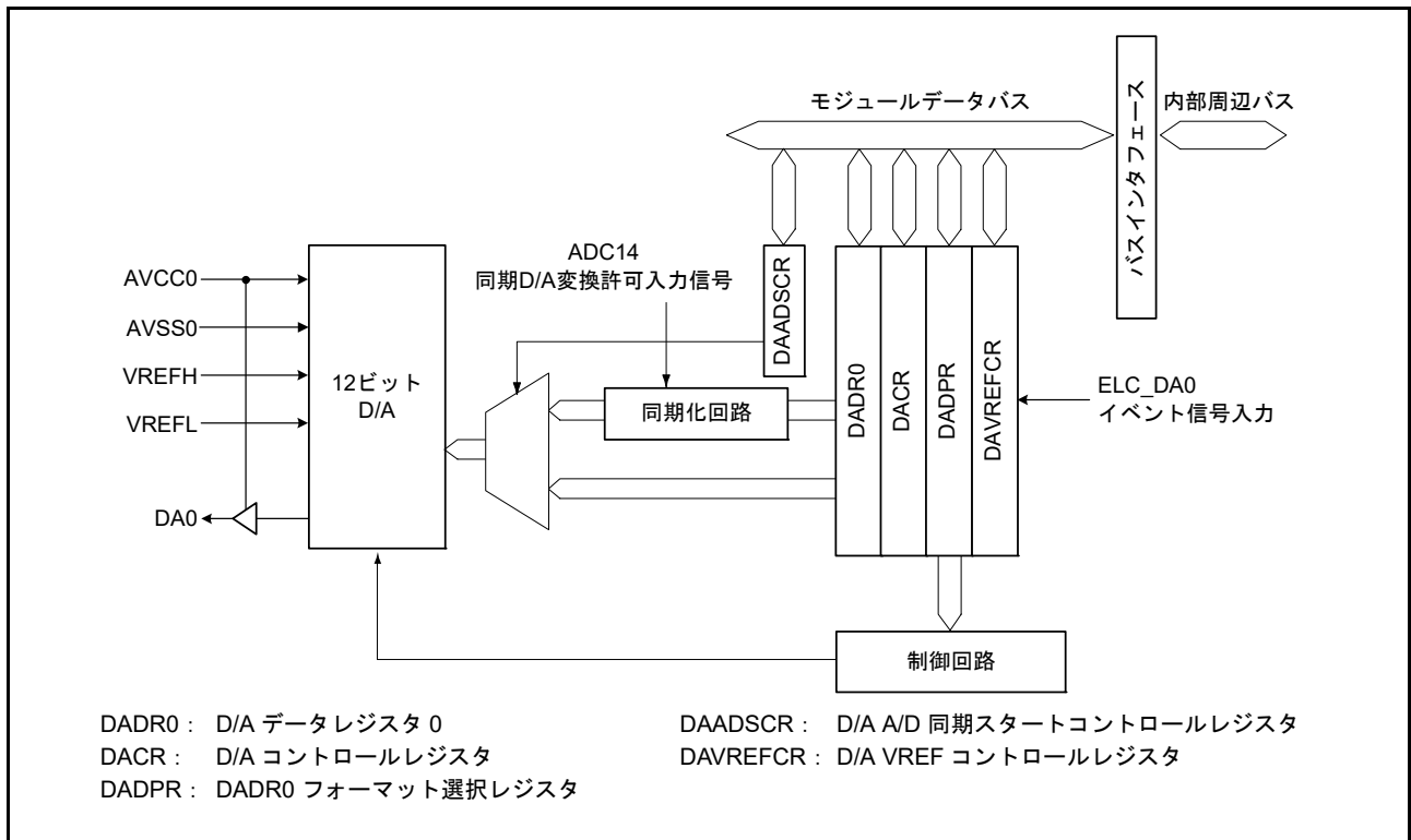
図 36.1 DAC12のブロック図
