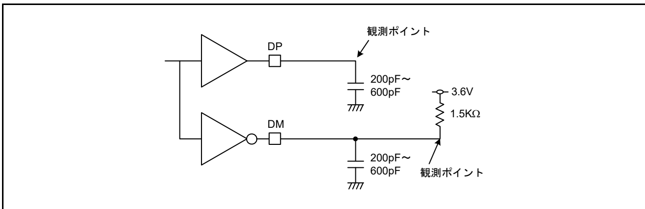
図 47.67 ロースピード (LS) 接続の測定回路
