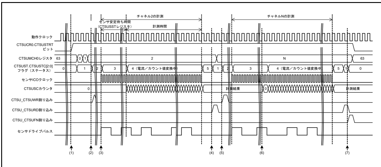
図 41.15 自己容量マルチスキャンモードのタイミング (計測開始条件がソフトウェアトリガの場合)
