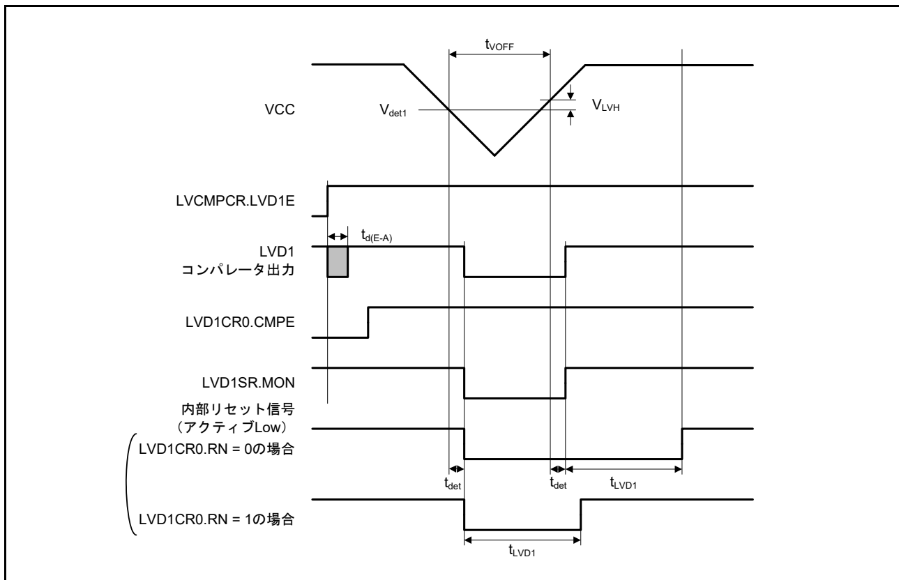
図 47.75 電圧検出回路タイミング ( V_{det1} )
