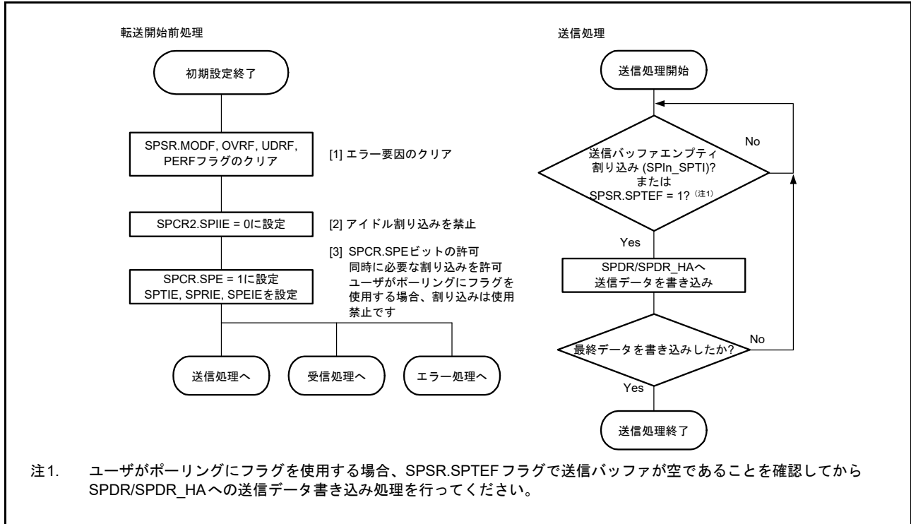
図 31.40 スレーブモードでの送信フロー
