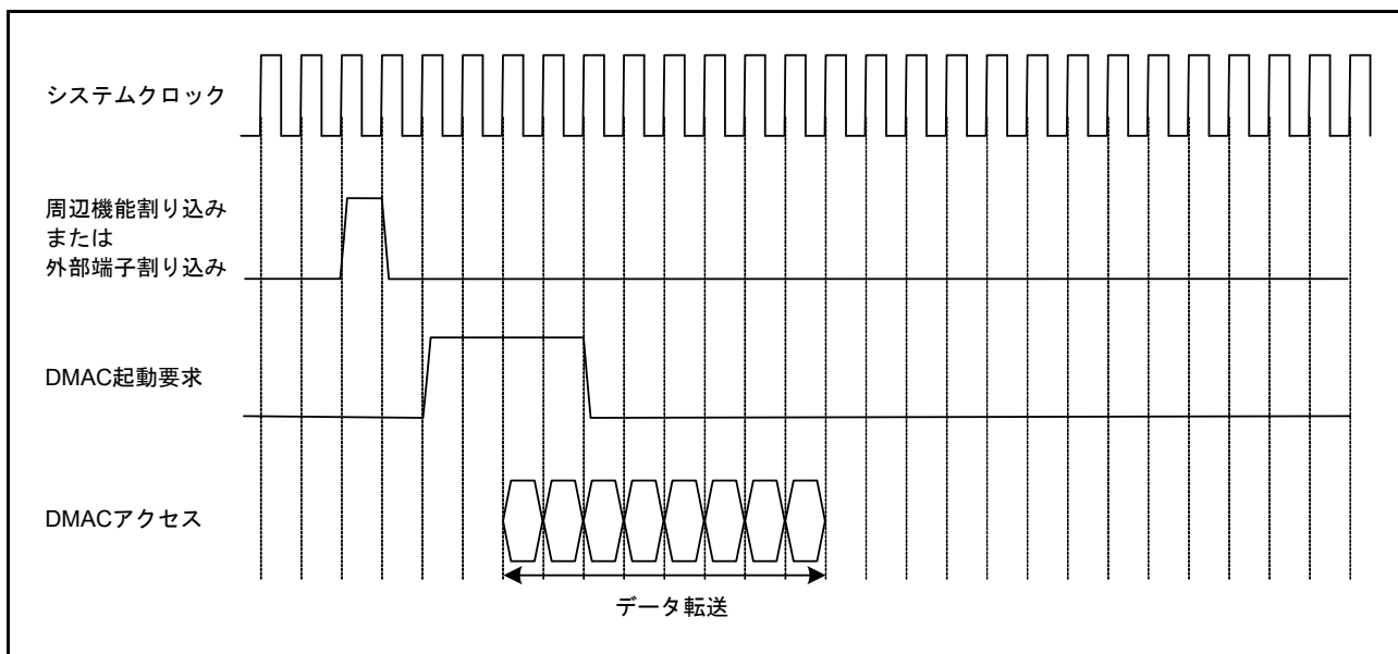
図 16.11 DMAC 動作タイミング例 2 (ブロックサイズ = 4 のブロック転送モードでの周辺モジュール/外部割り込み入力端子からの割り込みによる DMA 起動)
