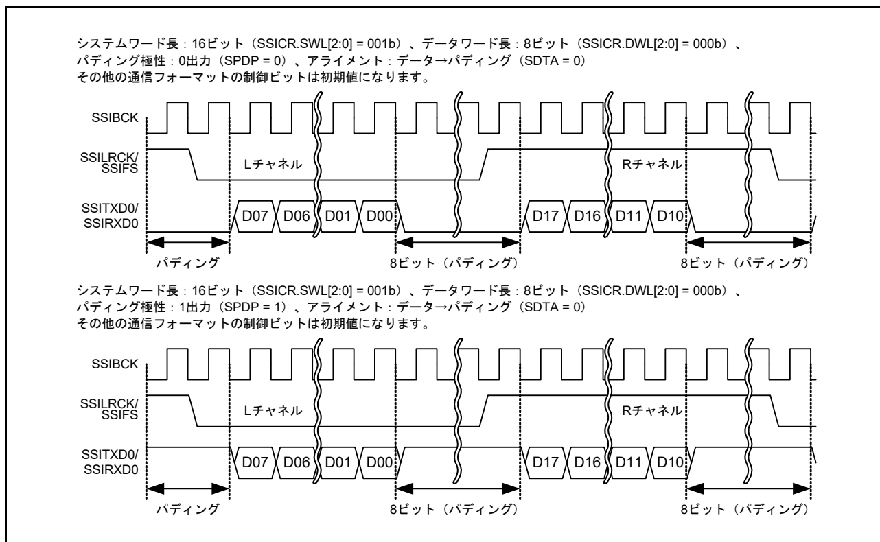
図 33.10 パディングビット極性
