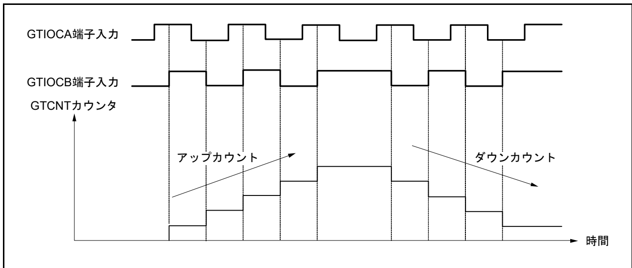
図 22.74 位相計数モード4 動作例
