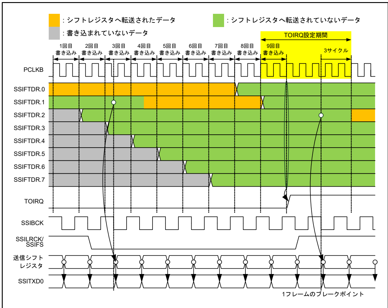
図 33.16 TOIRQ 設定タイミング
