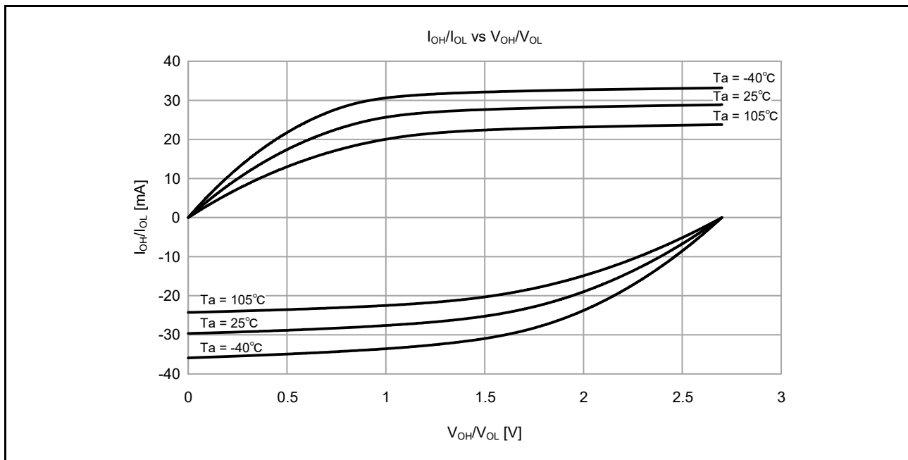
図 47.9 中駆動出力選択時の VCC = 2.7V での V OH /V OL および I OH /I OL 温度特性 (参考データ)
