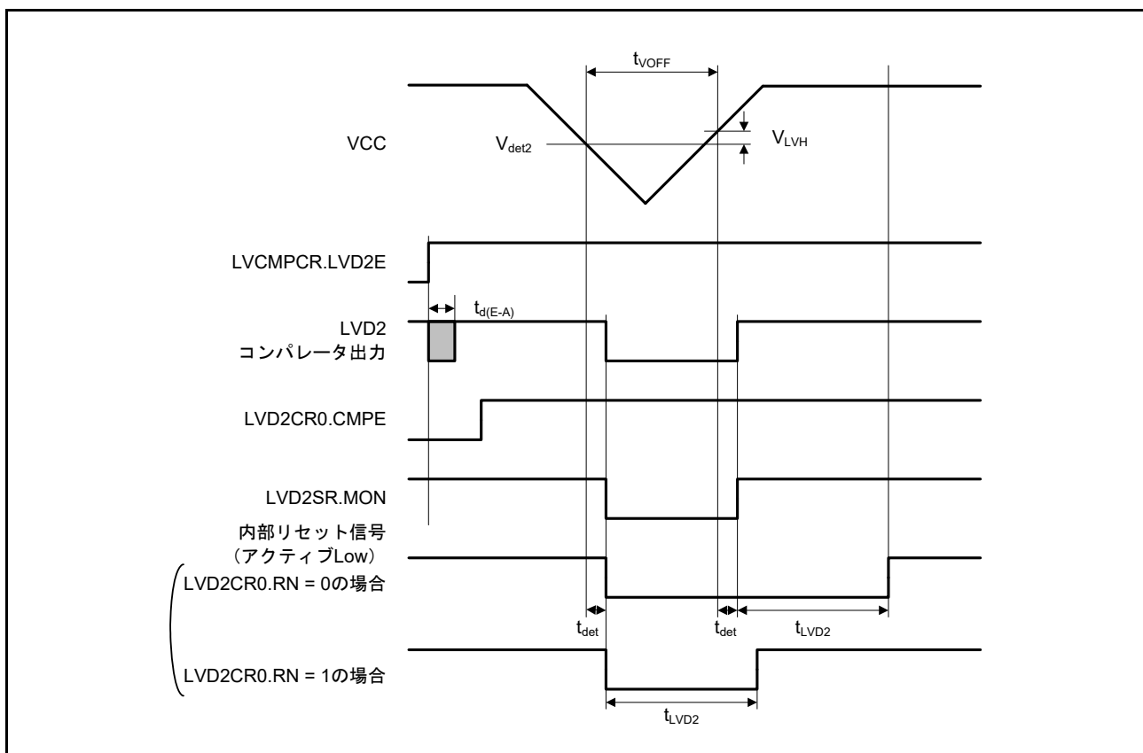
図 47.76 電圧検出回路タイミング ( V_{det2} )
