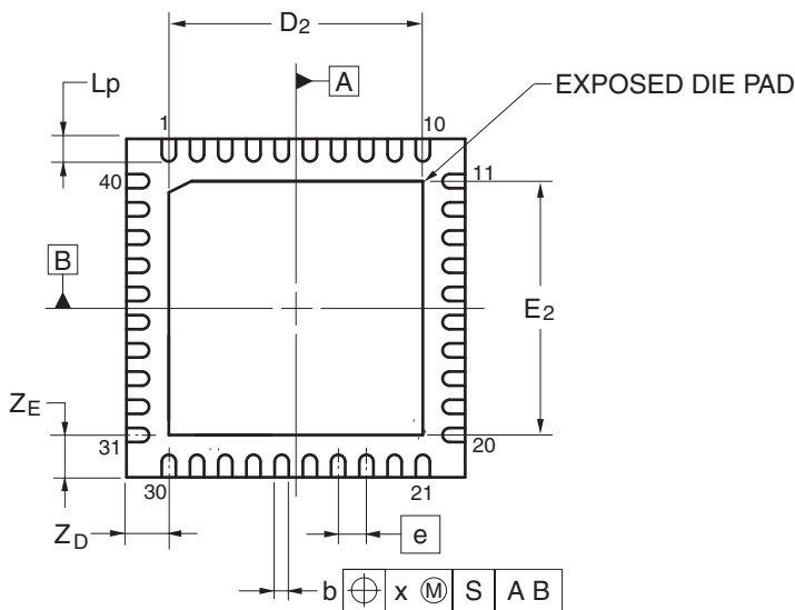
図 2.7 40-pin QFN
