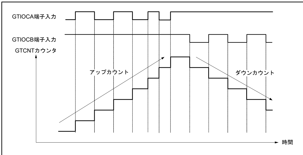
図 22.73 位相計数モード3 動作例 (C)
