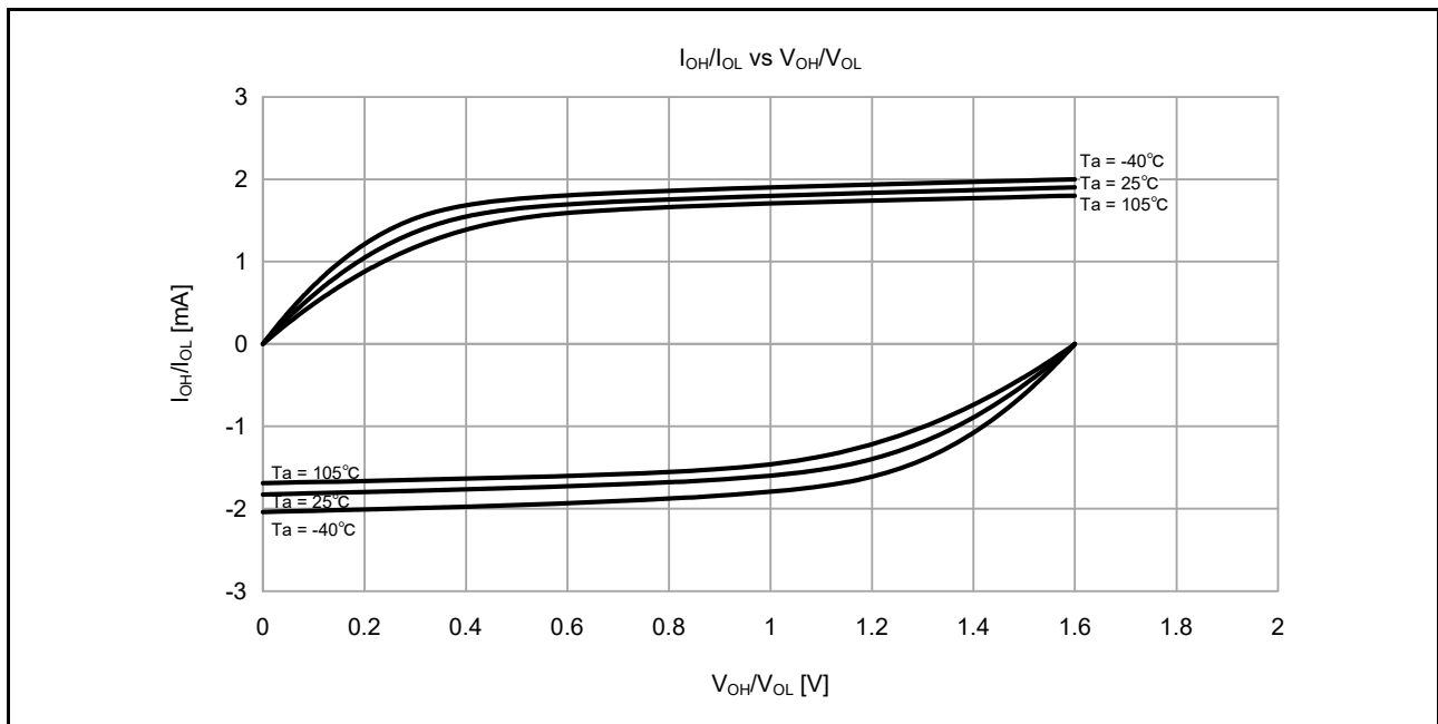
図 47.3 低駆動出力選択時の V_{CC} = 1.6V での V_{OH}/V_{OL} および I_{OH}/I_{OL} 温度特性 (参考データ)
