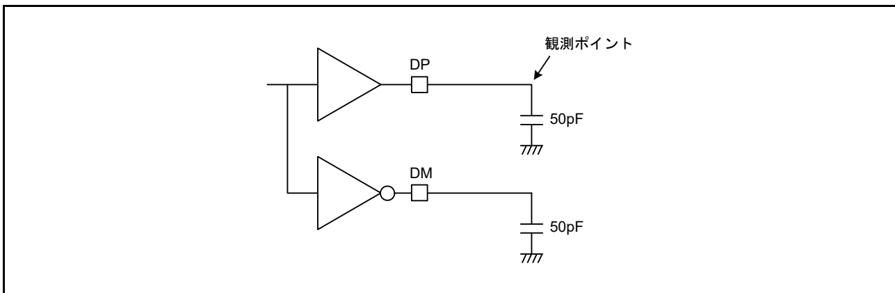
図 47.66 フルスピード (FS) 接続の測定回路
