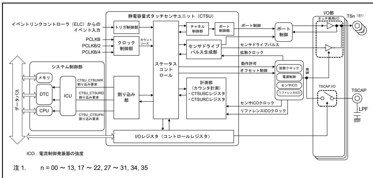
図 41.3 CTSUSのブロック図
