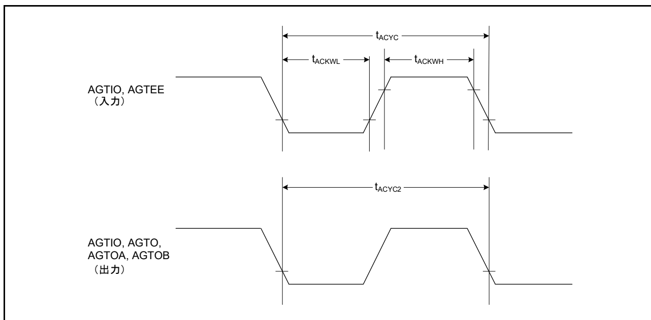
図 47.41 AGT 入出力タイミング
