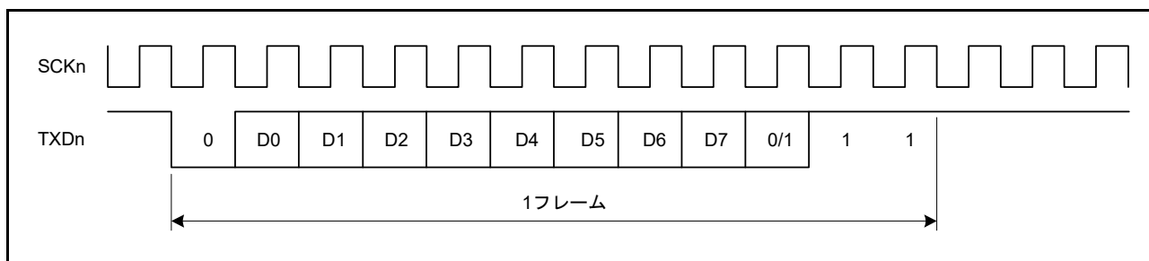
図 28.4 出力クロックと送信データの位相関係 (調歩同期式モード : SMR.CHR = 0、PE = 1、MP = 0、STOP = 1)
