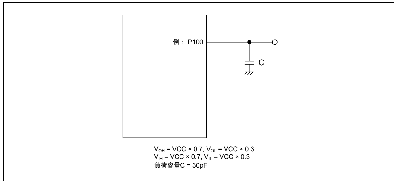
図 47.1 入出力タイミング計測条件
