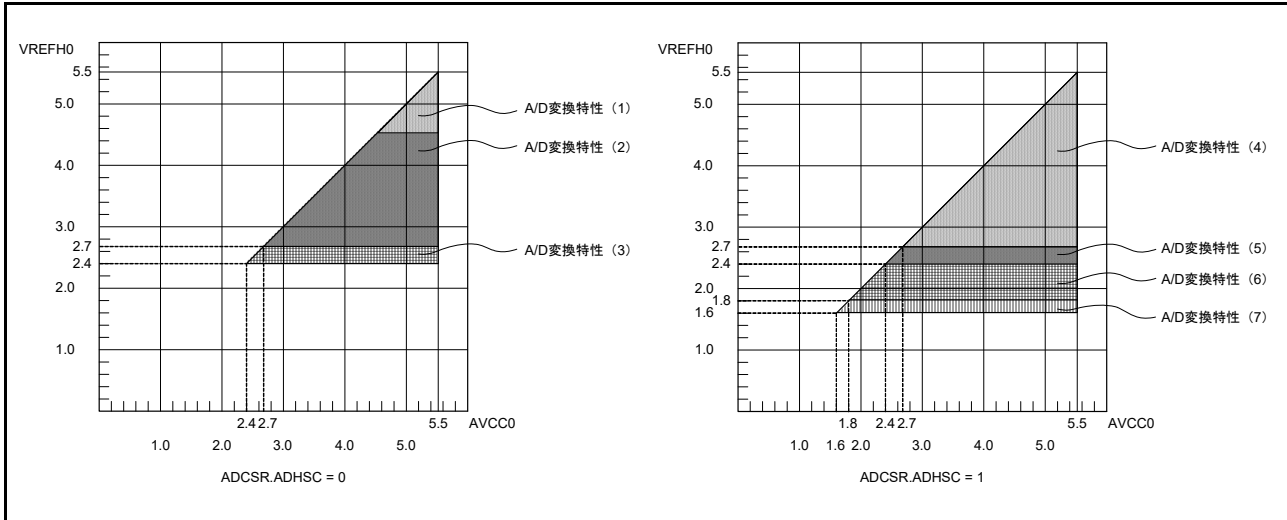
図 47.68 AVCC0 ~ VREFH0 電圧範囲
