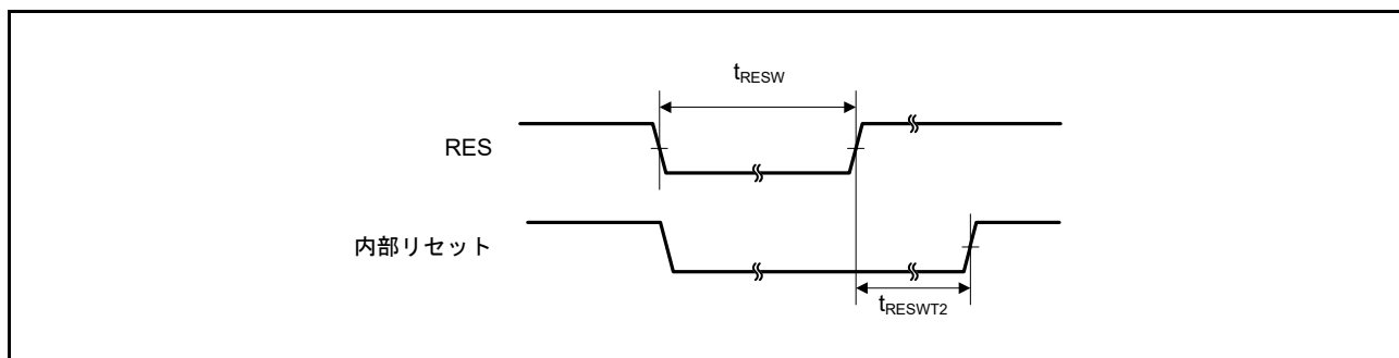
図 47.33 リセット入力タイミング
