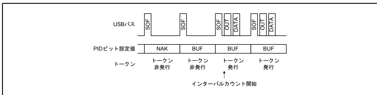
図 27.17 IITV = 0 の場合のトークン発行
