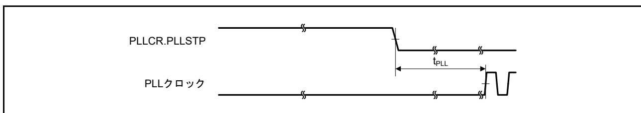
図 47.29 PLL クロック発振開始タイミング (メインクロックの発振安定後に PLL を動作させたとき)
