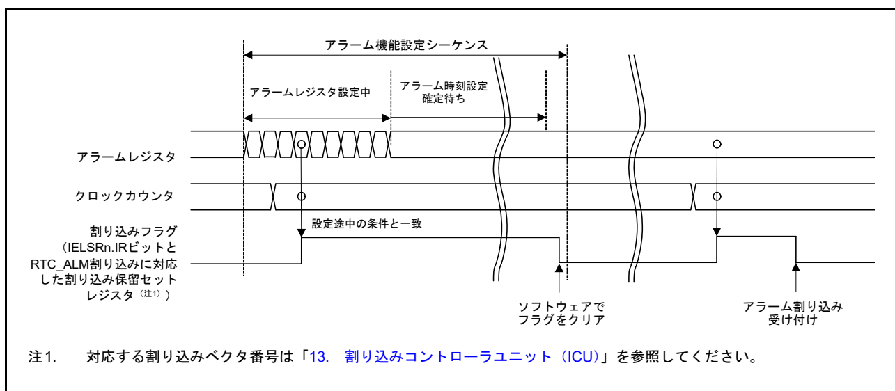
図 24.11 アラーム割り込み (RTC_ALM) のタイミング図
