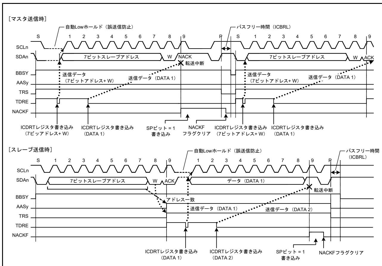
図 29.39 NACK 受信時のデータ転送中断動作 (NACKC = 1 の場合)
