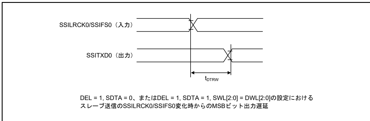
図 47.63 SSILRCK0/SSIFS0 変化時からの SSIE データ出力遅延
