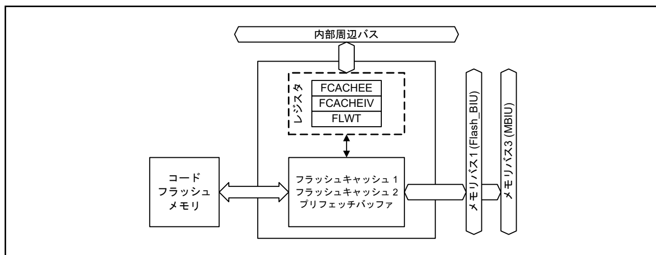
図 44.4 FCACHE のブロック図
