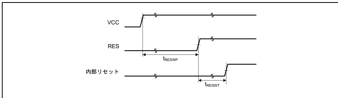
図 47.32 電源投入時リセット入力タイミング
