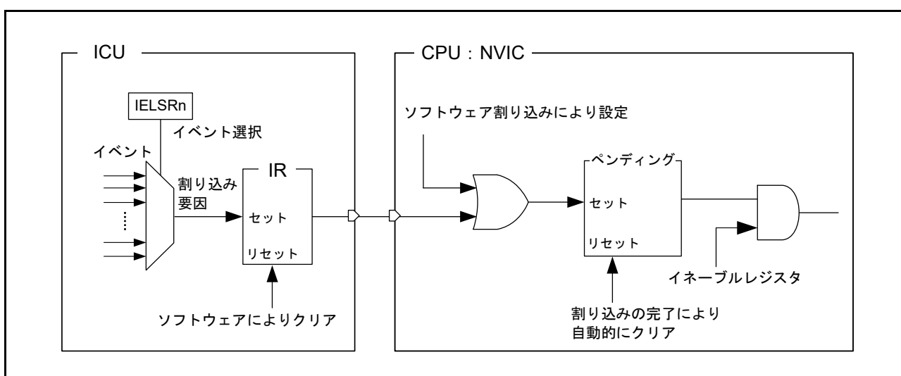
図 13.2 ICU および CPU: NVIC の割り込み経路
