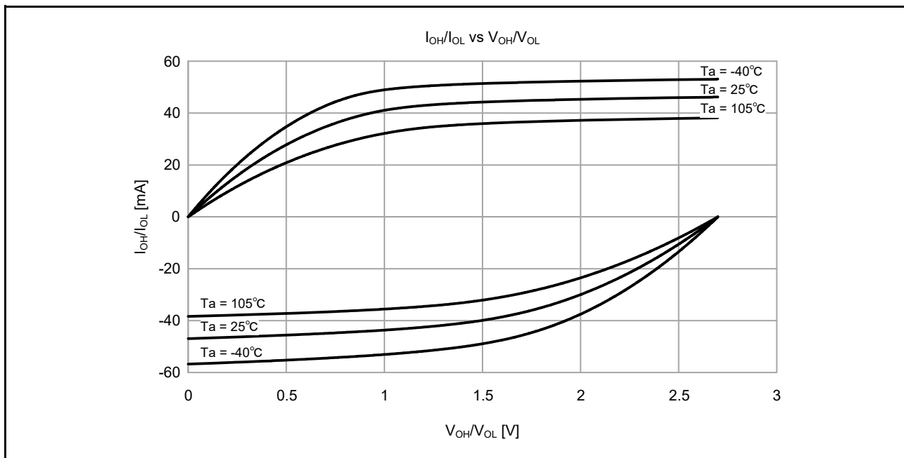
図 47.13 中駆動出力選択時の VCC = 2.7V での V OH /V OL および I OH /I OL 温度特性 (参考データ)
