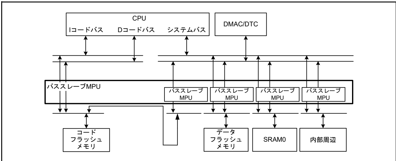
図 15.9 バススレーブ MPU のブロック図
