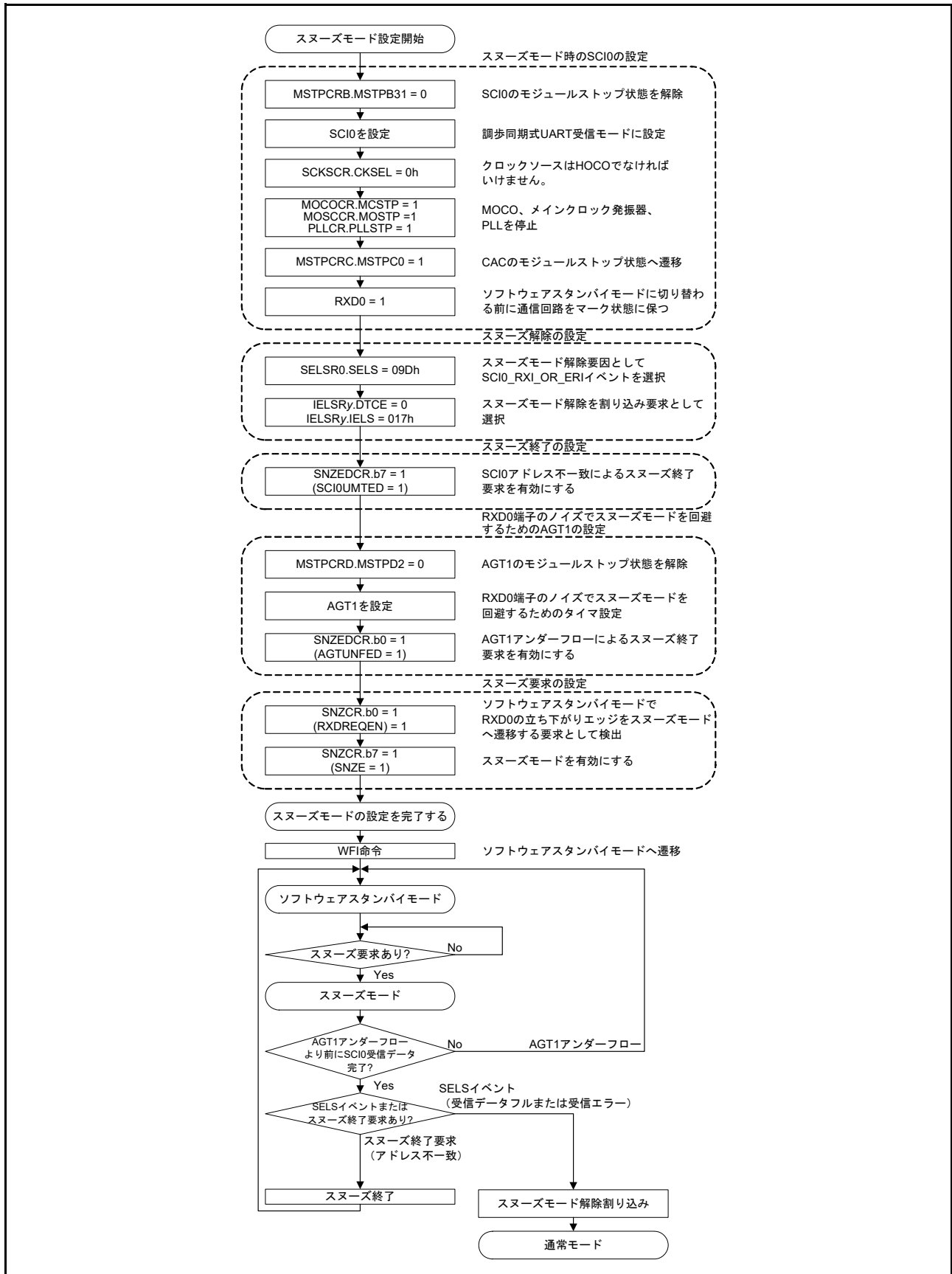
図 10.12 スヌーズモードエントリで SCIO を使用するための設定例
