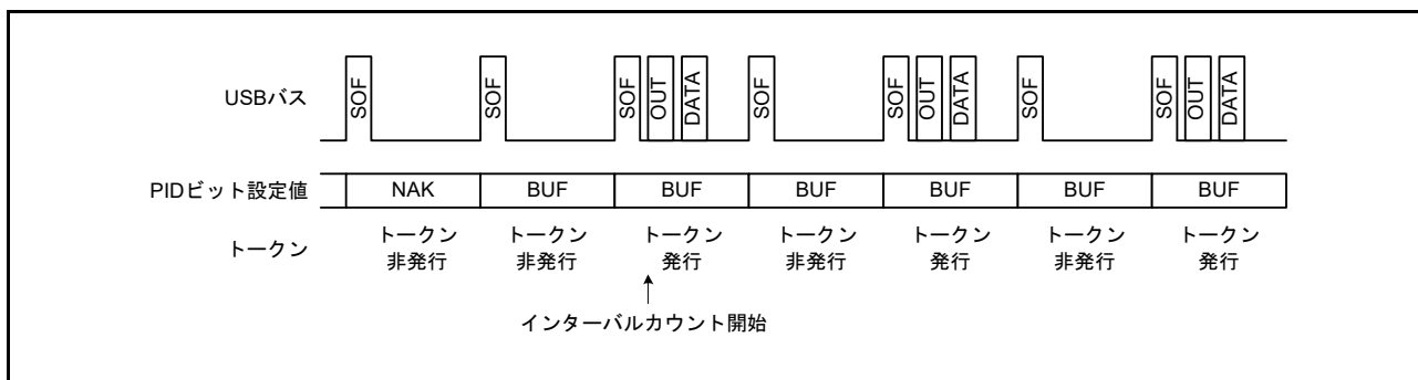
図 27.18 IITV = 1 の場合のトークン発行
