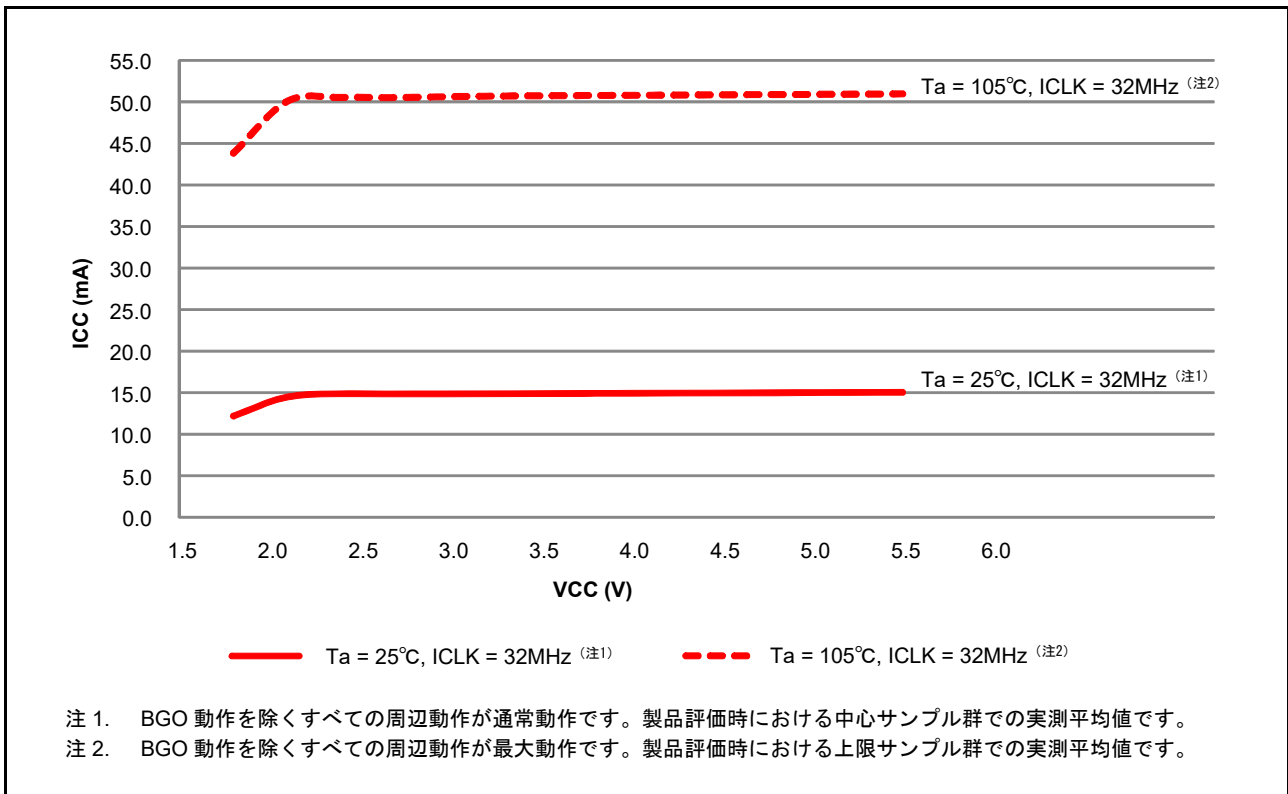
図 47.21 Subosc-speed モードにおける電圧依存性 (参考データ)
