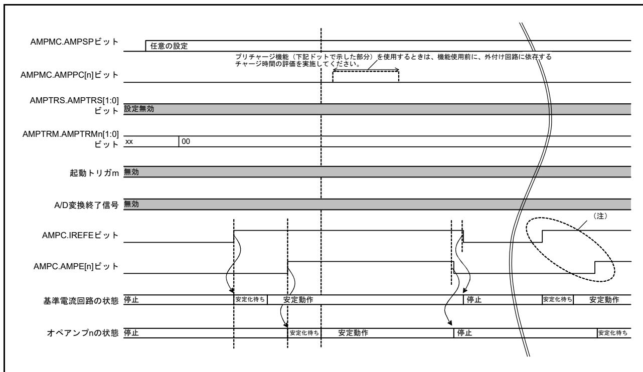
図 38.3 オペアンプの制御動作 (ソフトウェアトリガモードによる制御) (ソフトウェアトリガモードによって標準電流回路およびオペアンプを起動/停止する場合)
