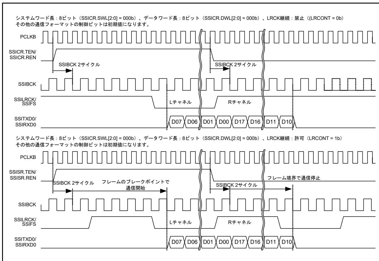
図 33.31 LR クロック/フレーム同期継続の動作例
