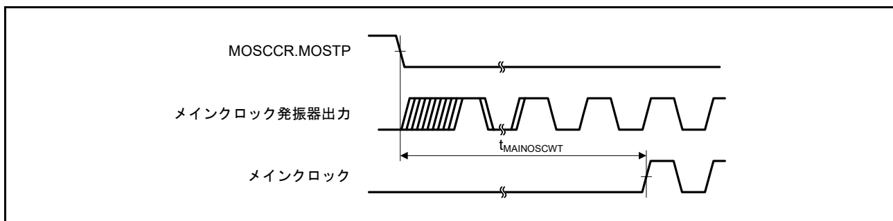
図 47.28 メインクロック発振開始タイミング
