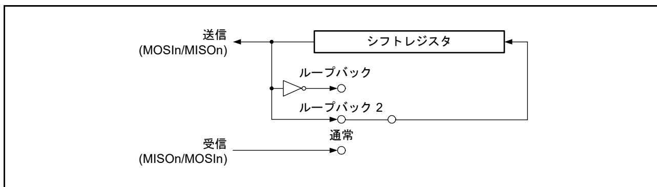
図 31.48 ループバックモード時のシフトレジスタ入出力経路の構成 (マスターモード)
