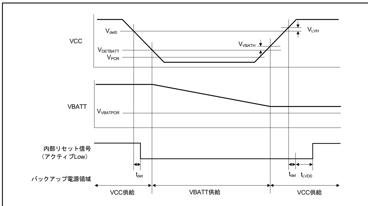
図 47.77 電源切り替えおよび LVD0 リセットタイミング
