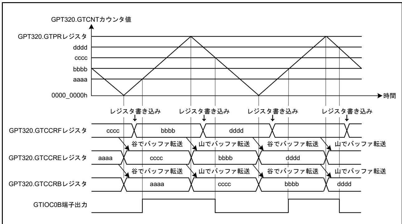
図 22.24 GTCCRA、GTCCRB レジスタのダブルバッファ動作例 (アウトプットコンペア、三角波、山と谷でバッファ動作、GTCCRB レジスタのコンペアマッチでトグル出力、周期の終わりで出力保持の場合)
