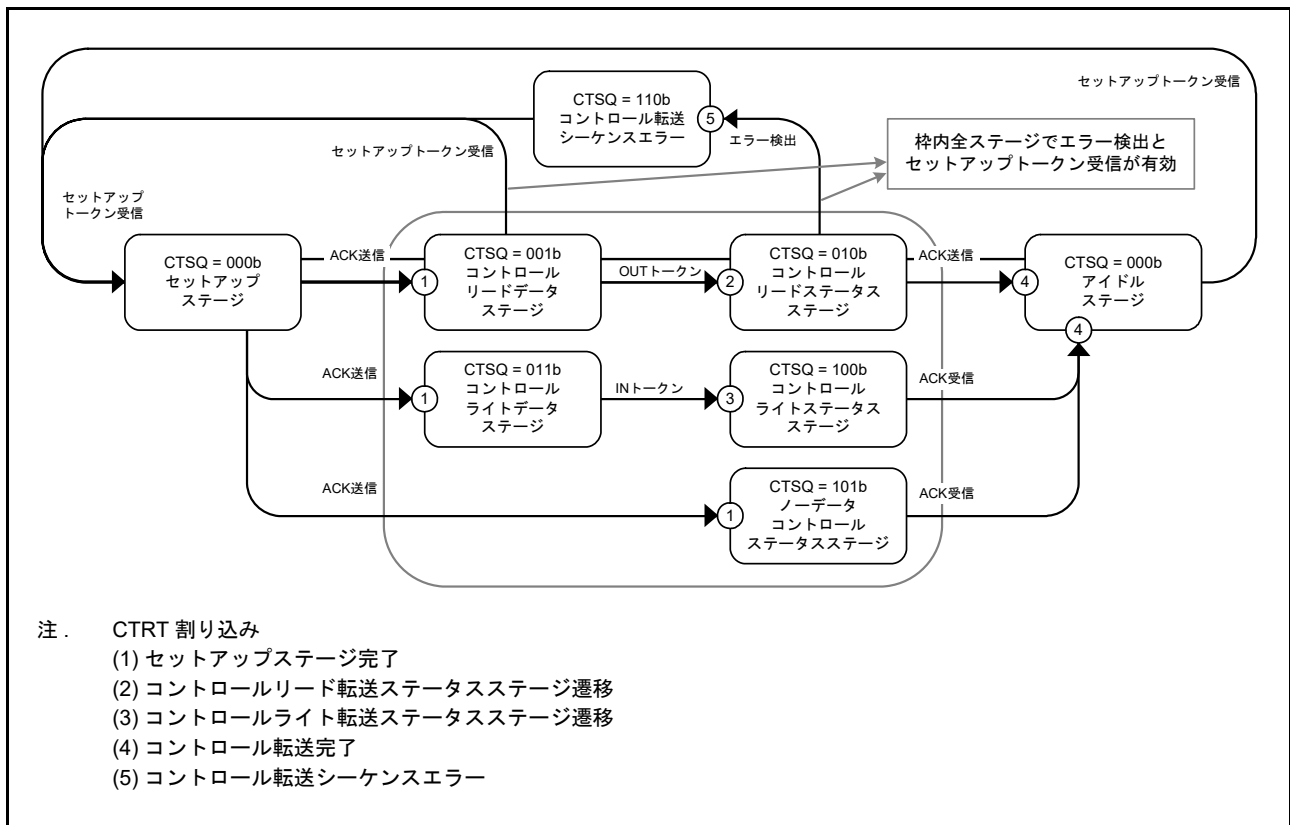
図 27.16 コントロール転送ステージの遷移
