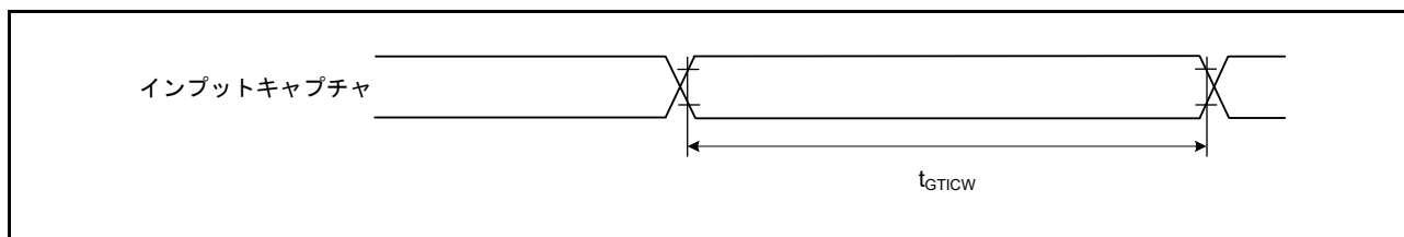
図 47.40 GPT インプットキャプチャタイミング
