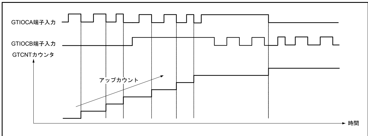
図 22.75 位相計数モード5 動作例 (A)
