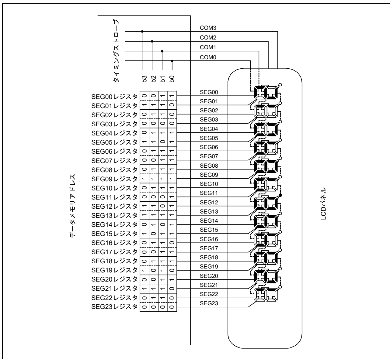
図 45.29 4 時分割 LCD パネルの接続例
