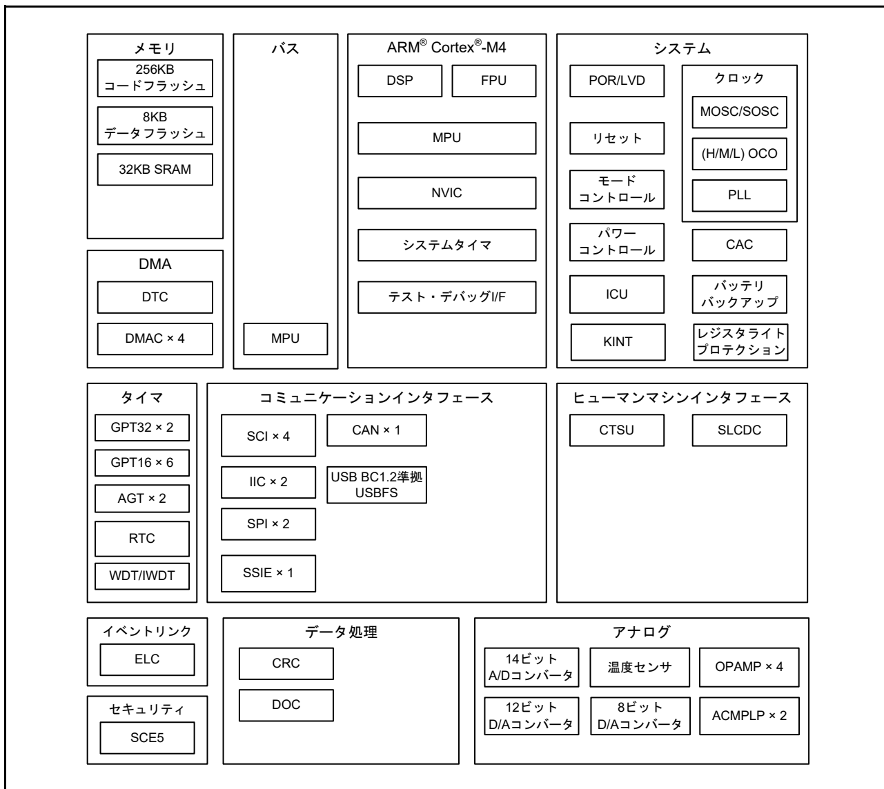
図 1.1 ブロック図
