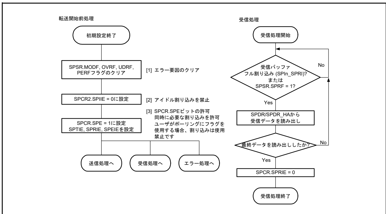
図 31.41 スレーブモードでの受信フロー
