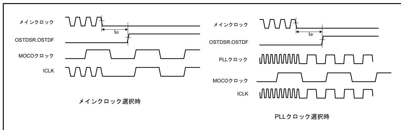
図 47.71 発振停止検出タイミング
