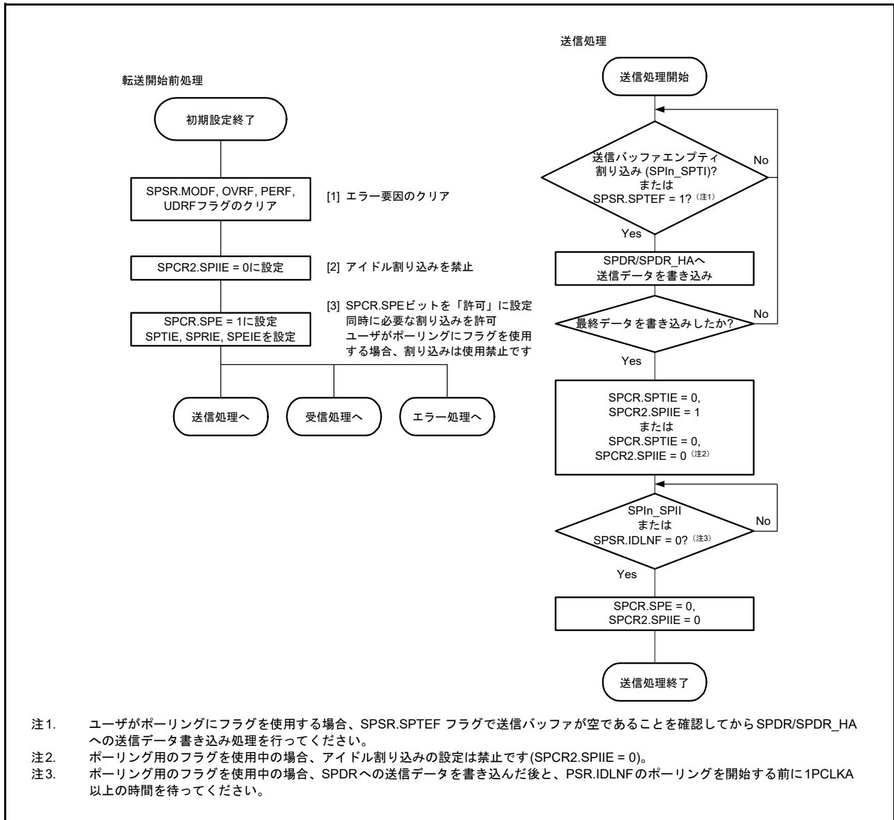
図 31.36 マスタモードでの送信フロー
