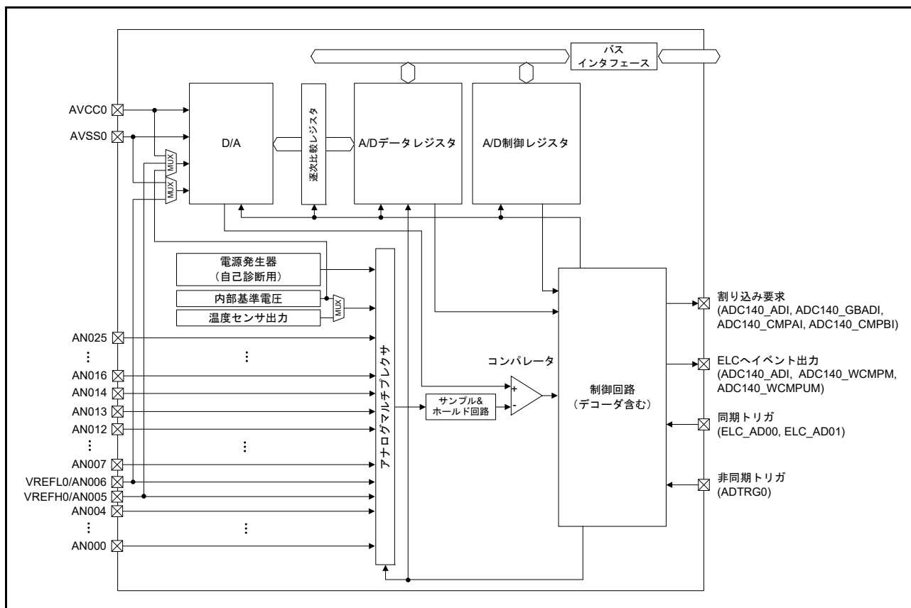
図 35.1 ADC14のブロック図
