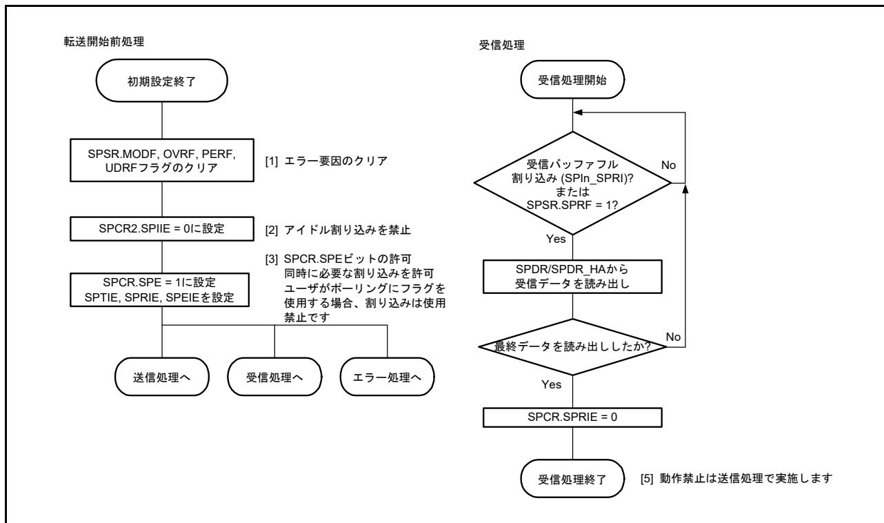
図 31.37 マスタモードでの受信フロー
