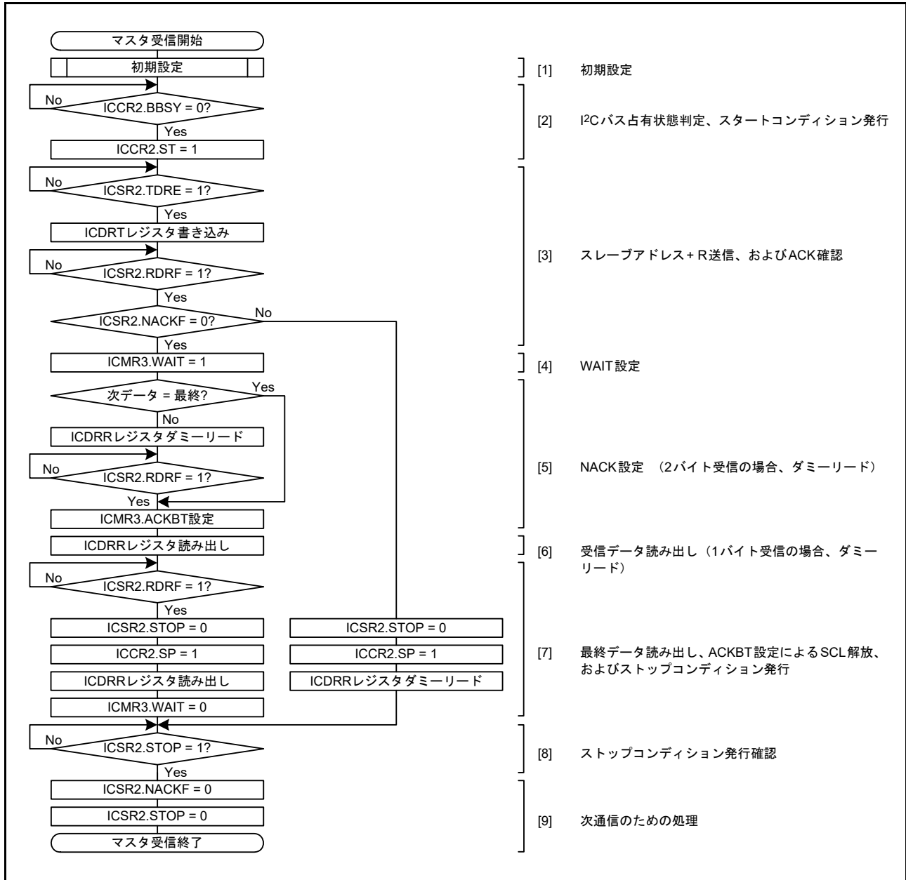
図 29.10 マスタ受信の例 (7ビットアドレスフォーマット、1~2バイト受信時)
