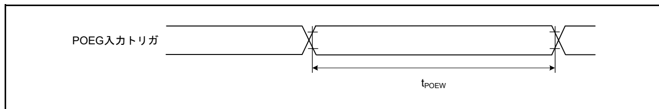
図 47.39 POEG 入カトリガタイミング
