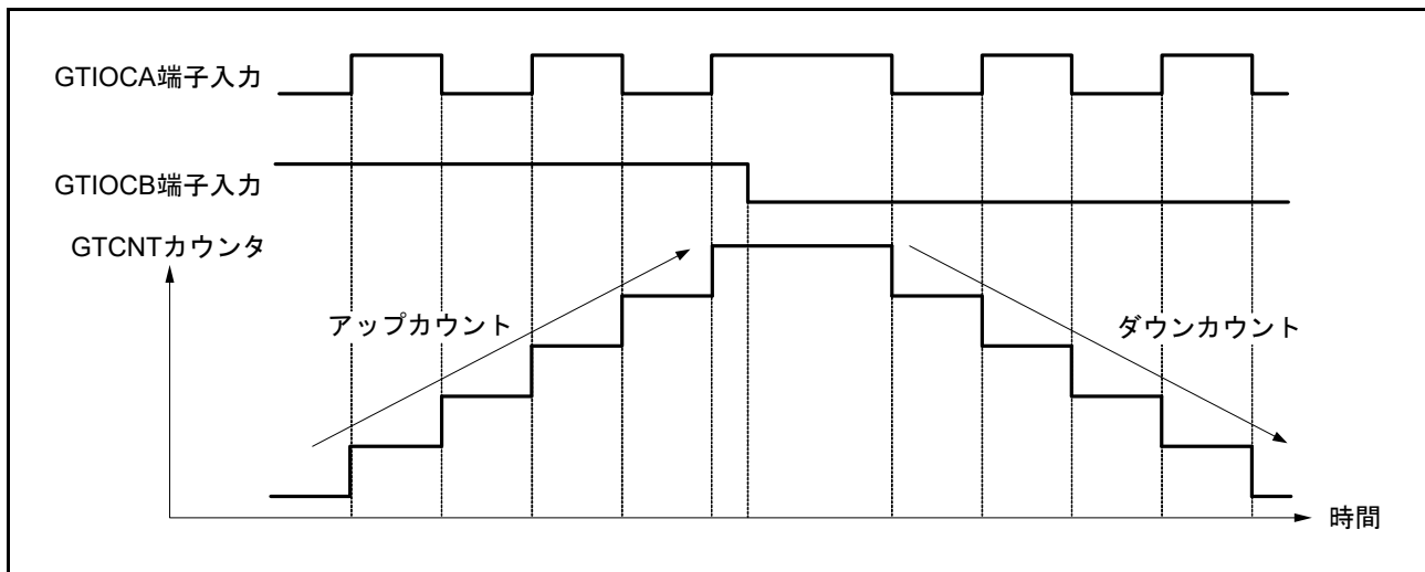
図 22.70 位相計数モード2 動作例 (C)
