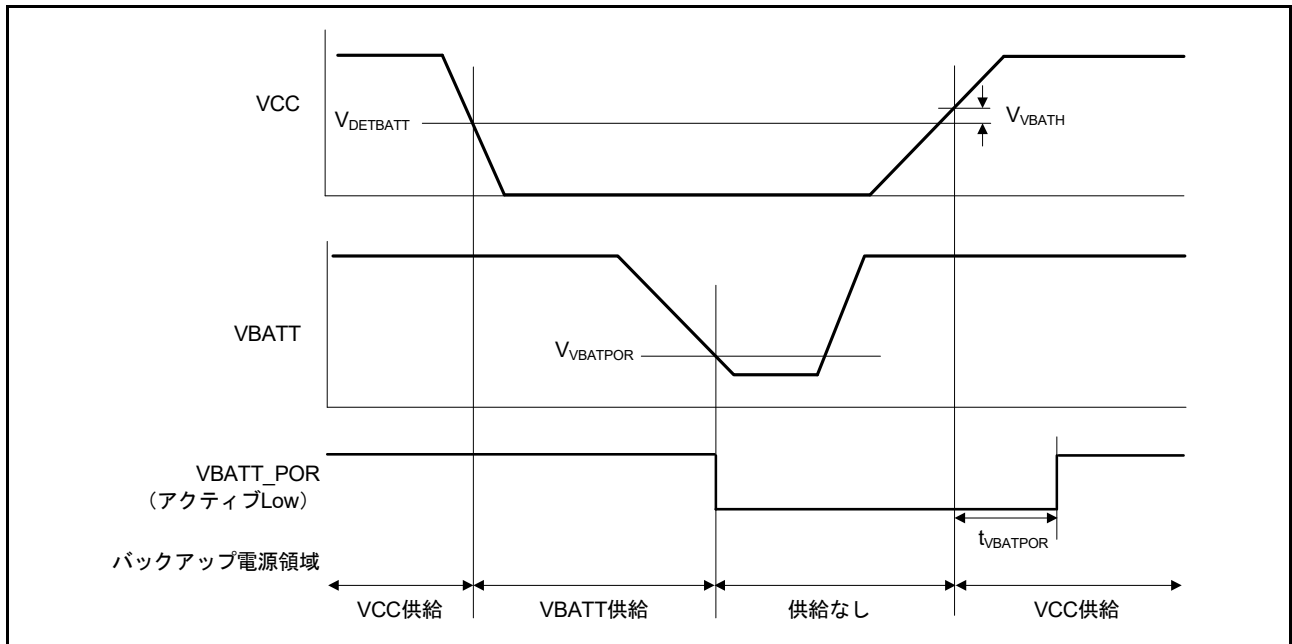
図 47.78 VBATT_POR リセットタイミング
