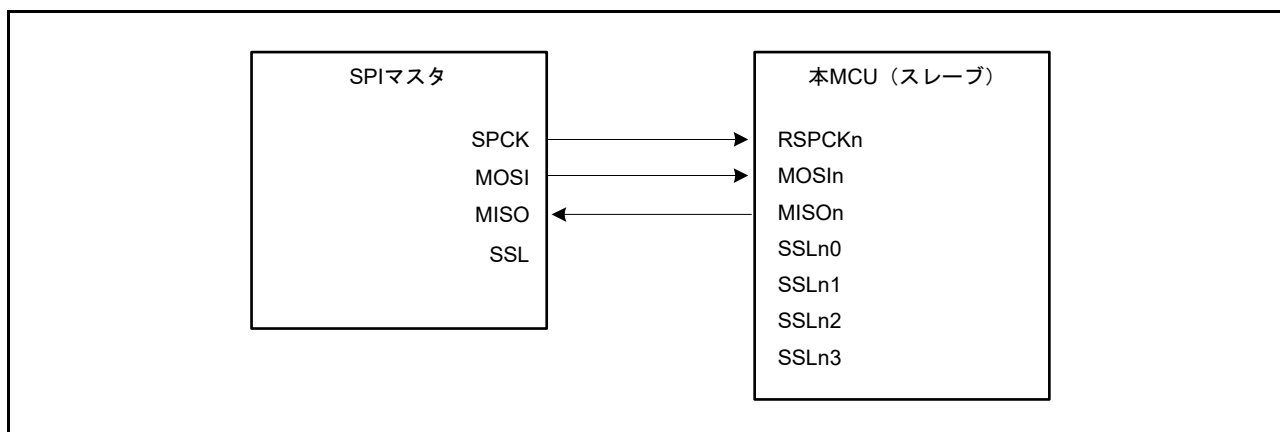
図 31.12 クロック同期モードのマスター/スレーブの構成例 (MCU はスレーブ、CPHA = 1)
