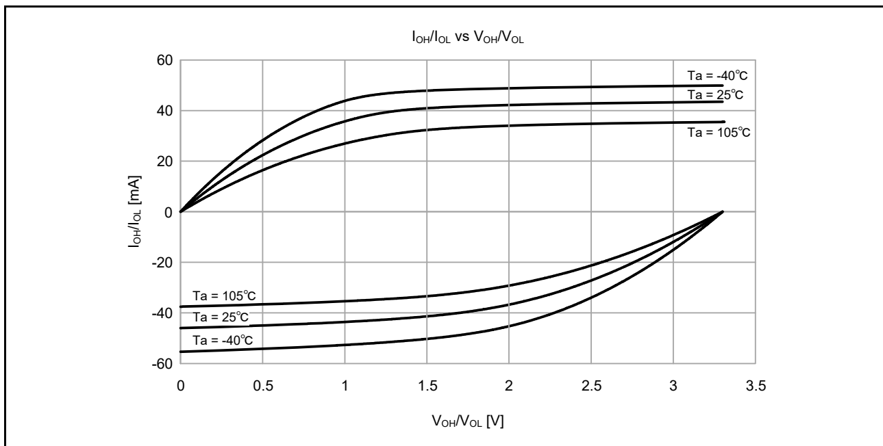
図 47.10 中駆動出力選択時の VCC = 3.3V での V OH /V OL および I OH /I OL 温度特性 (参考データ)
