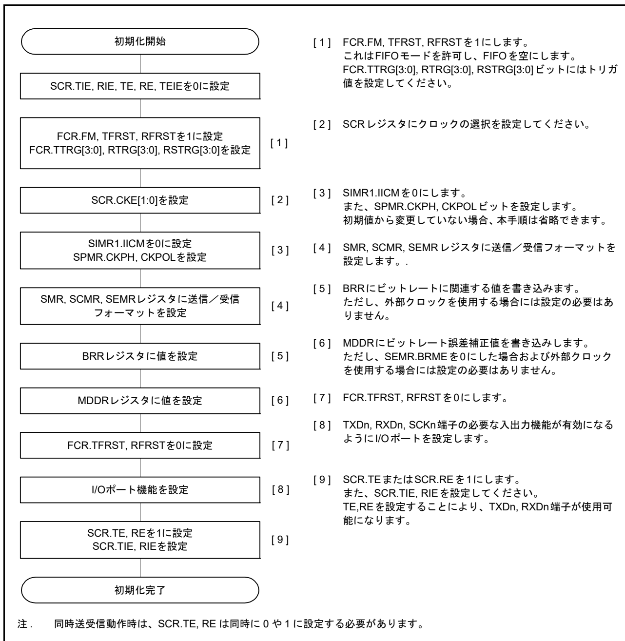
図 28.33 クロック同期式モードにおける SCI の初期化フローチャート例 (FIFO 選択時)
