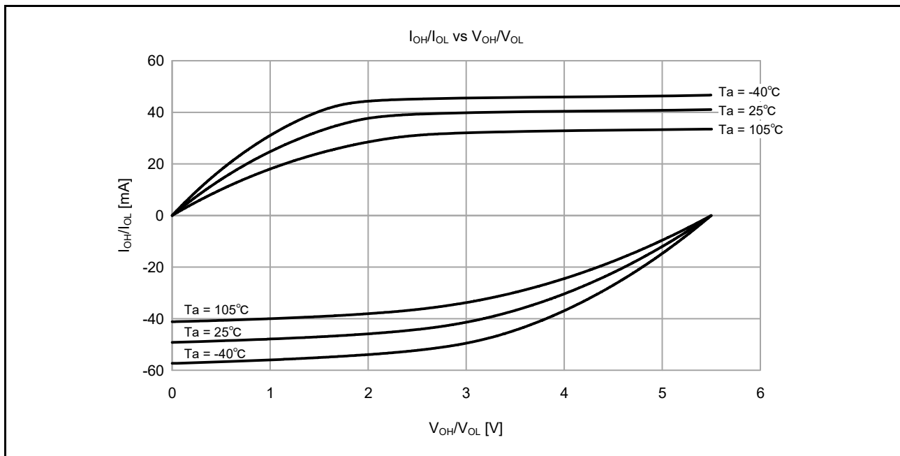
図 47.6 低駆動出力選択時の VCC = 5.5V での V_{OH}/V_{OL} および I_{OH}/I_{OL} 温度特性 (参考データ)
