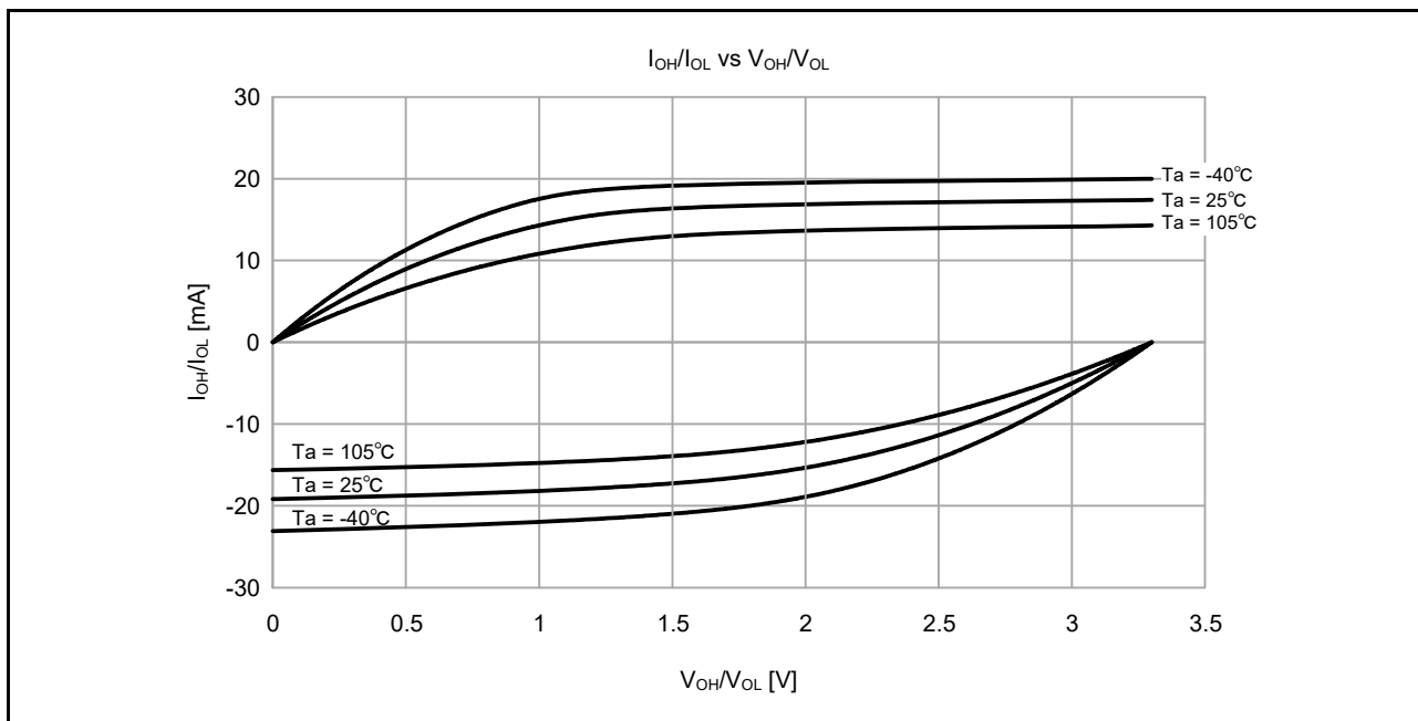
図 47.5 低駆動出力選択時の VCC = 3.3V での V_{OH}/V_{OL} および I_{OH}/I_{OL} 温度特性 (参考データ)
