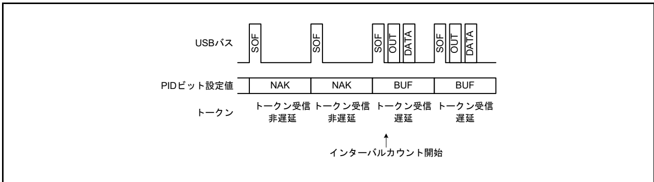
図 27.19 フレームとトークン受信待機の関係 (IITV = 0 の場合)
