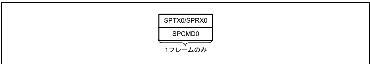
図 31.45 シーケンス動作時の SPI コマンドレジスタと送受信バッファの関係
