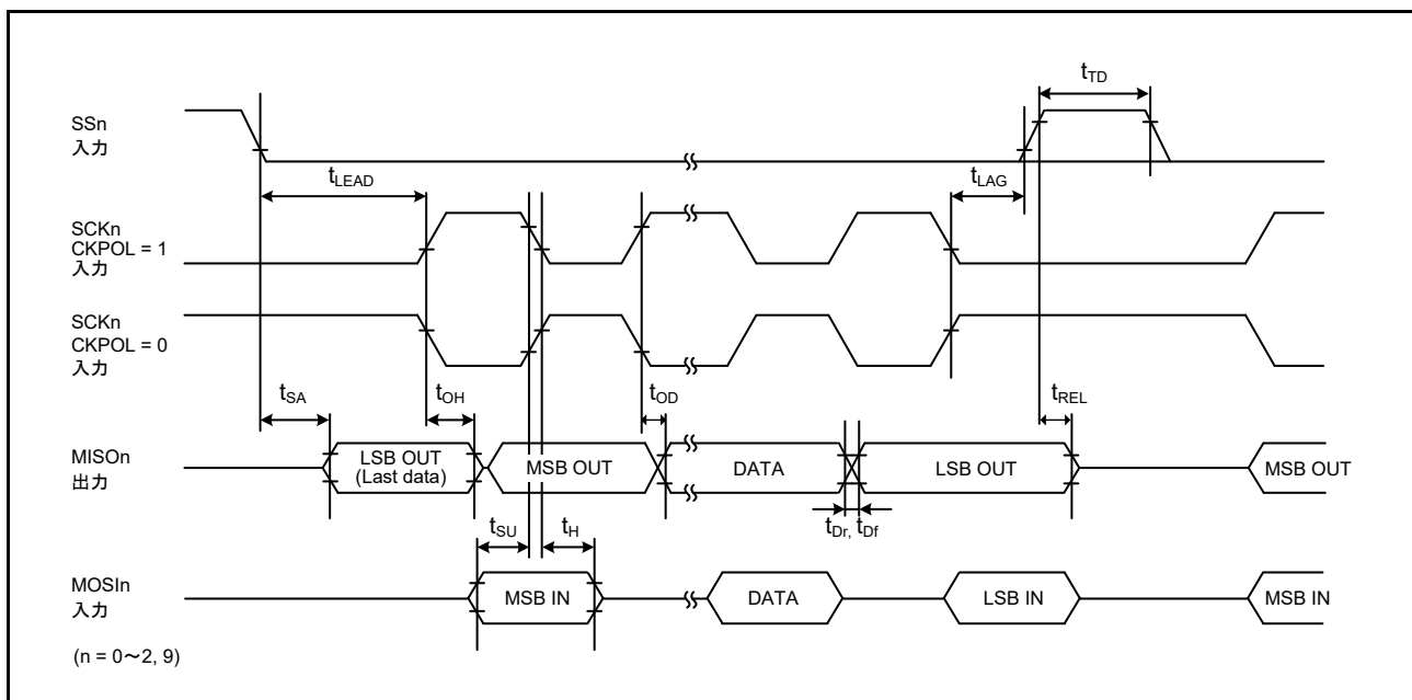
図 47.50 SCI 簡易 SPI モードタイミング (スレーブ、CKPH = 0)
