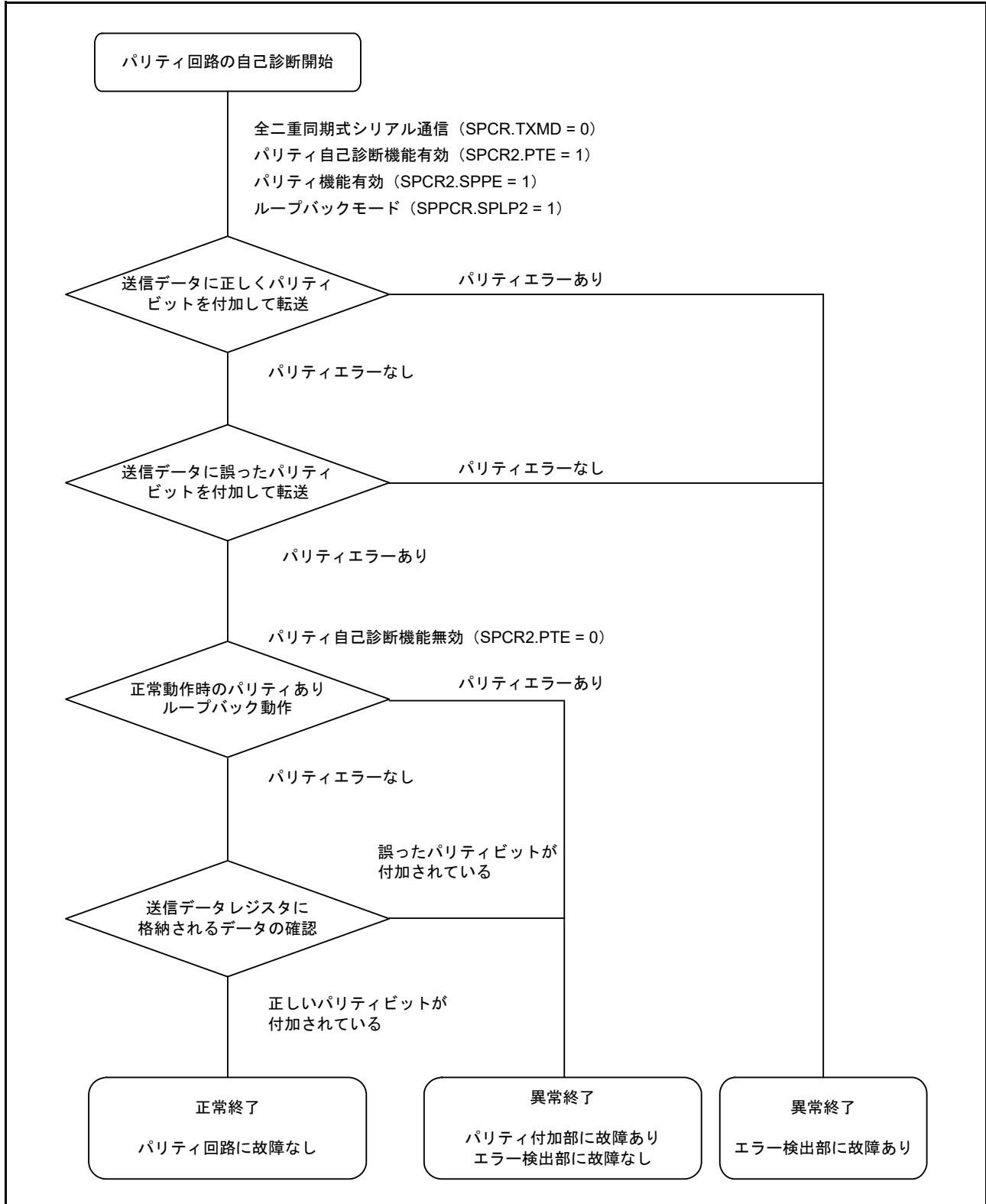
図 31.49 パリティ回路の自己診断フロー
