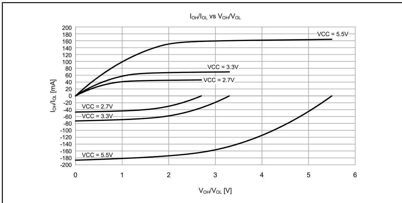
図 47.12 中駆動出力選択時の Ta = 25 °Cでの V OH /V OL および I OH /I OL 電圧特性 (参考データ)
