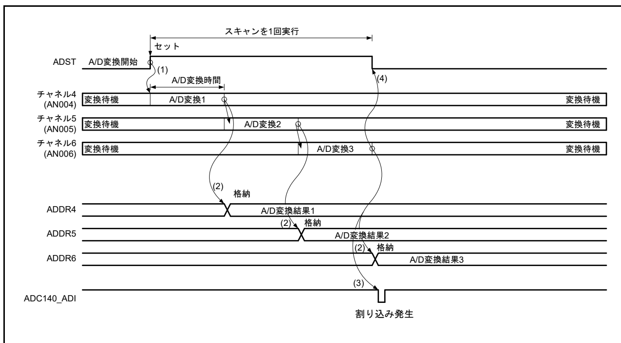
図 35.6 シングルスキャンモードの動作例 (基本動作 : AN004 ~ AN006 選択)
