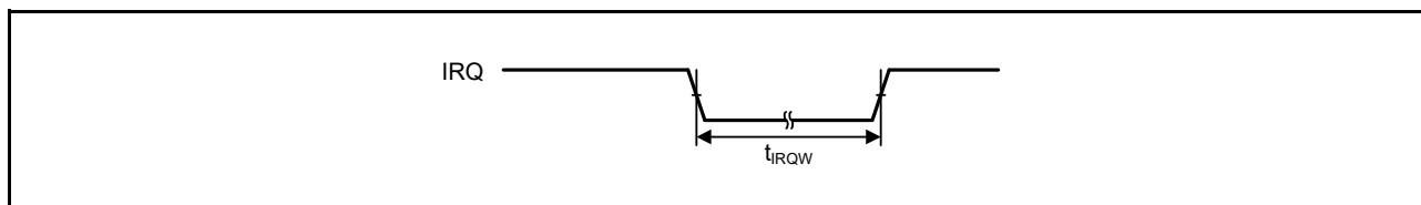
図 47.37 IRQ 割り込み入力タイミング
