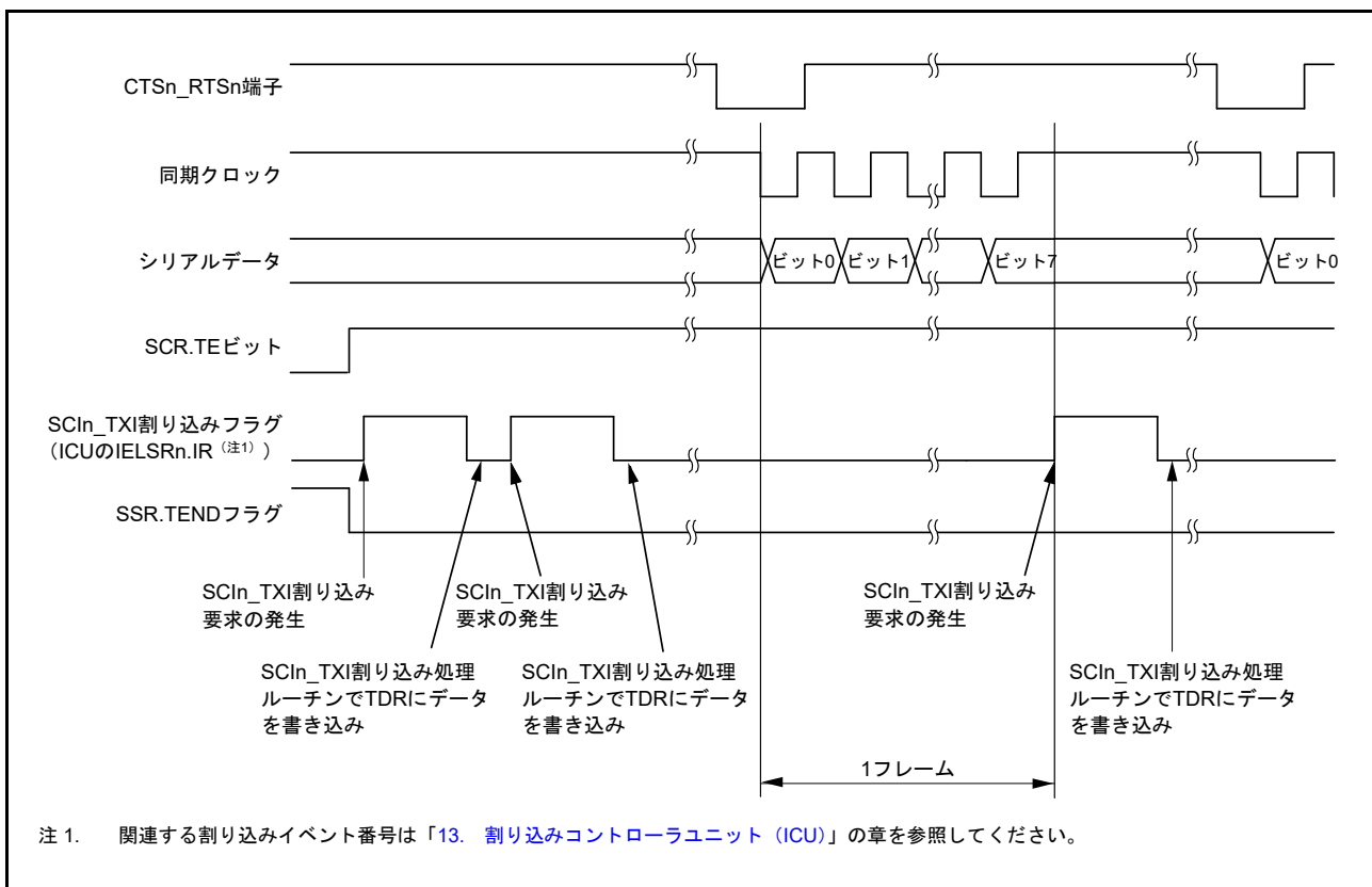
図 28.35 クロック同期式モードにおけるシリアル送信の動作例 (送信開始時に CTS 機能を使用する場合)
