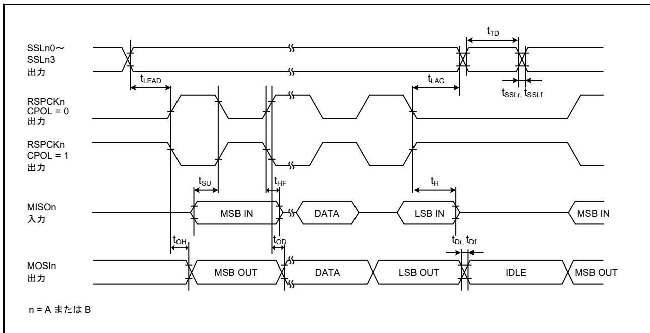
図 47.56 SPI タイミング (マスター、CPHA = 1) (ビットレート : PCLKA を 2 分周に設定)
