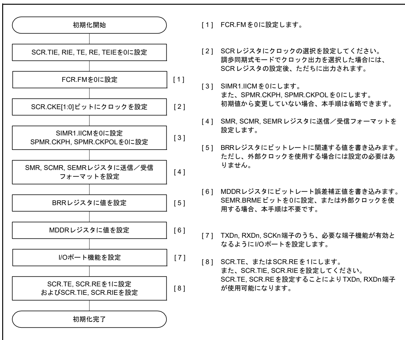
図 28.7 調歩同期式モードにおける SCI の初期化フローチャート例 (非 FIFO 選択時)
