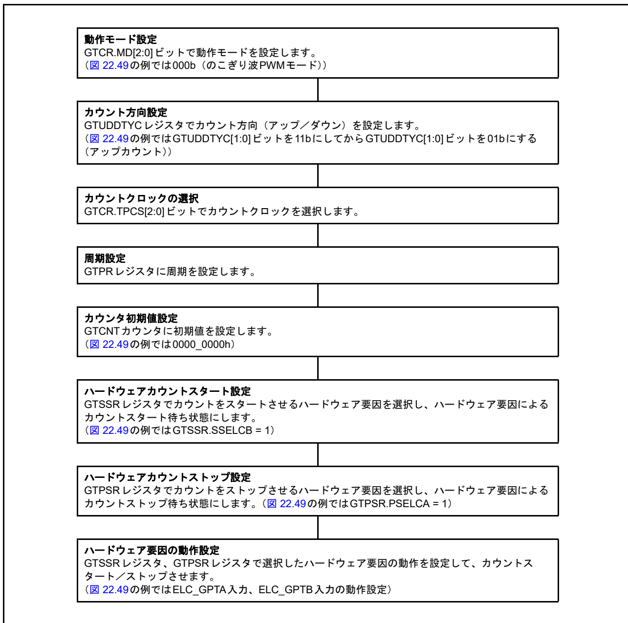
図 22.50 ハードウェア要因によるカウンタストップ動作設定例
