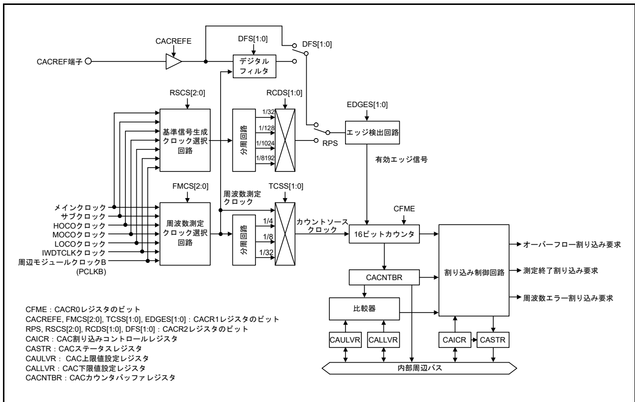
図 9.1 CAC のブロック図
