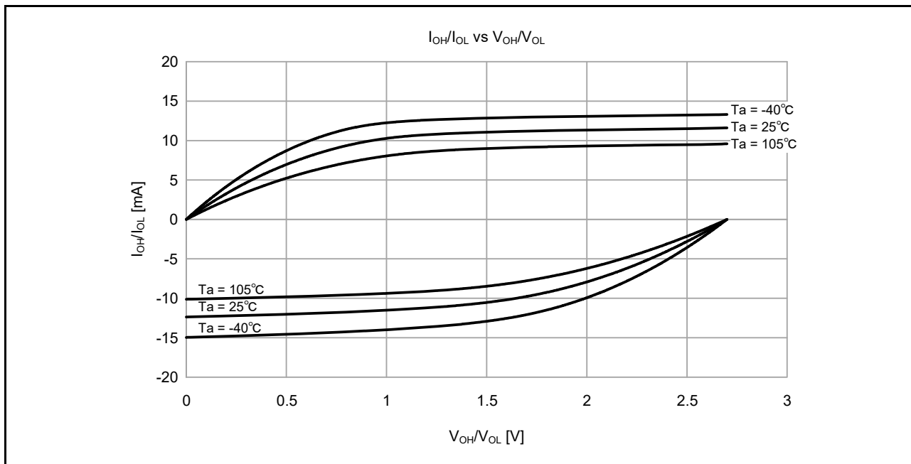
図 47.4 低駆動出力選択時の VCC = 2.7V での V_{OH}/V_{OL} および I_{OH}/I_{OL} 温度特性 (参考データ)
