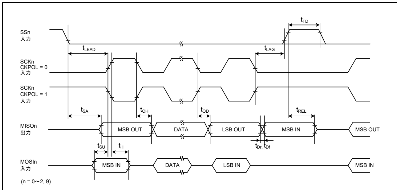
図 47.49 SCI 簡易 SPI モードタイミング (スレーブ、CKPH = 1)
