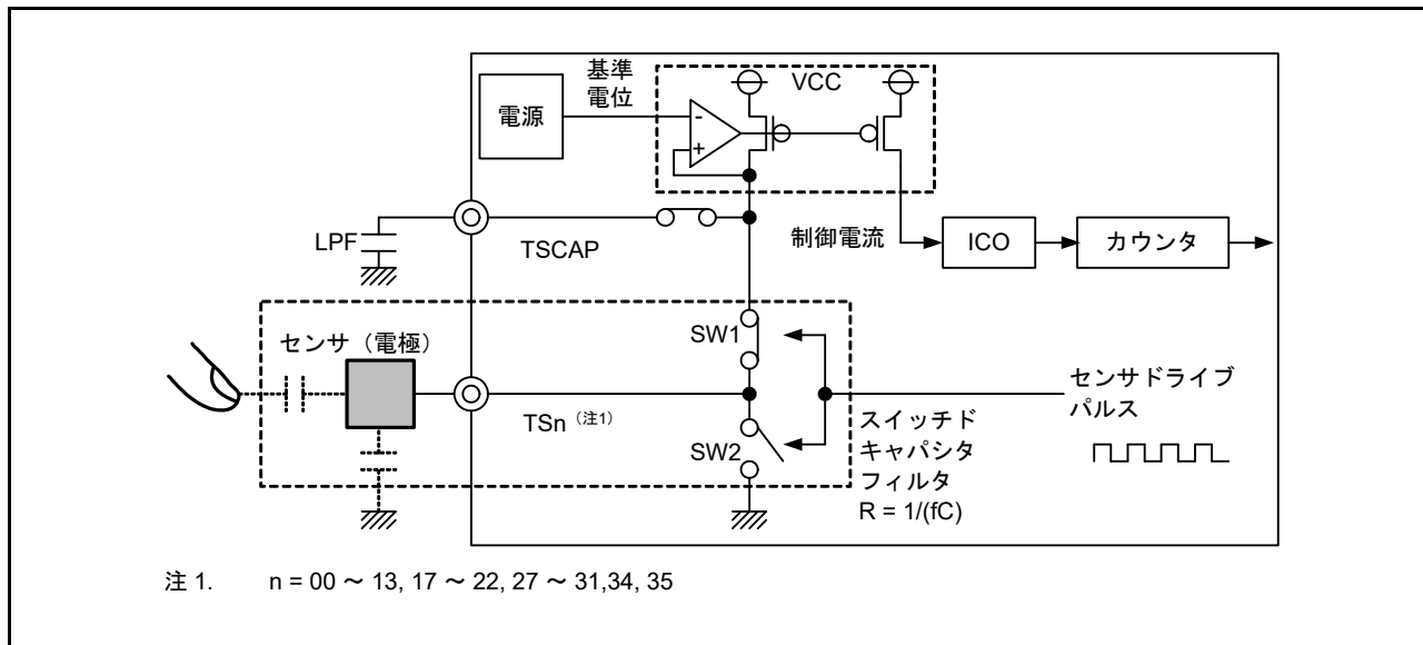
図 41.4 計測部回路
