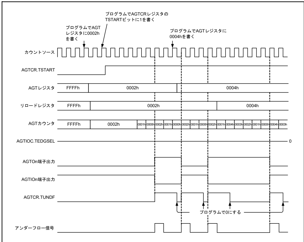
図 23.6 パルス出力モードでの動作例
