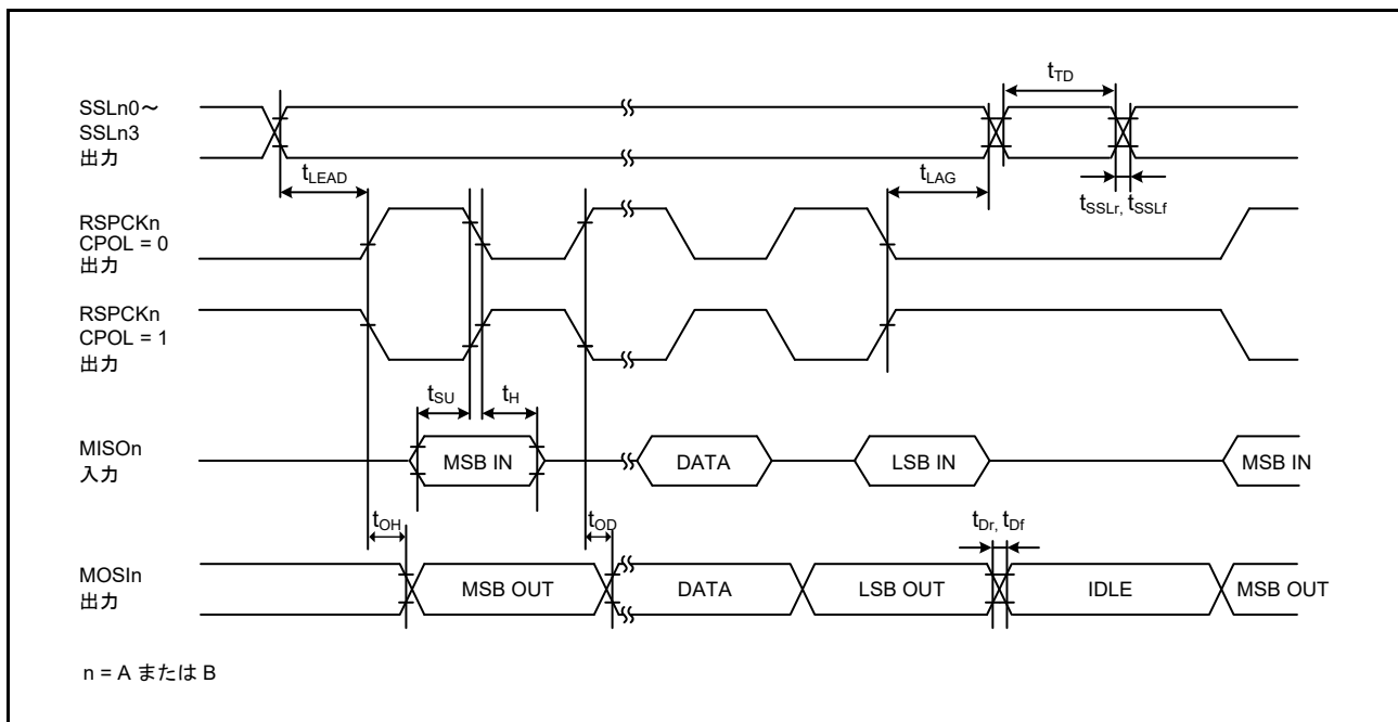
図 47.55 SPI タイミング (マスタ、CPHA = 1) (ビットレート : PCLKA を 2 分周以外に設定)
