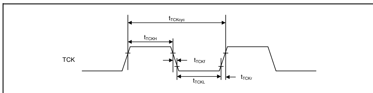
図 47.84 JTAG TCK タイミング
