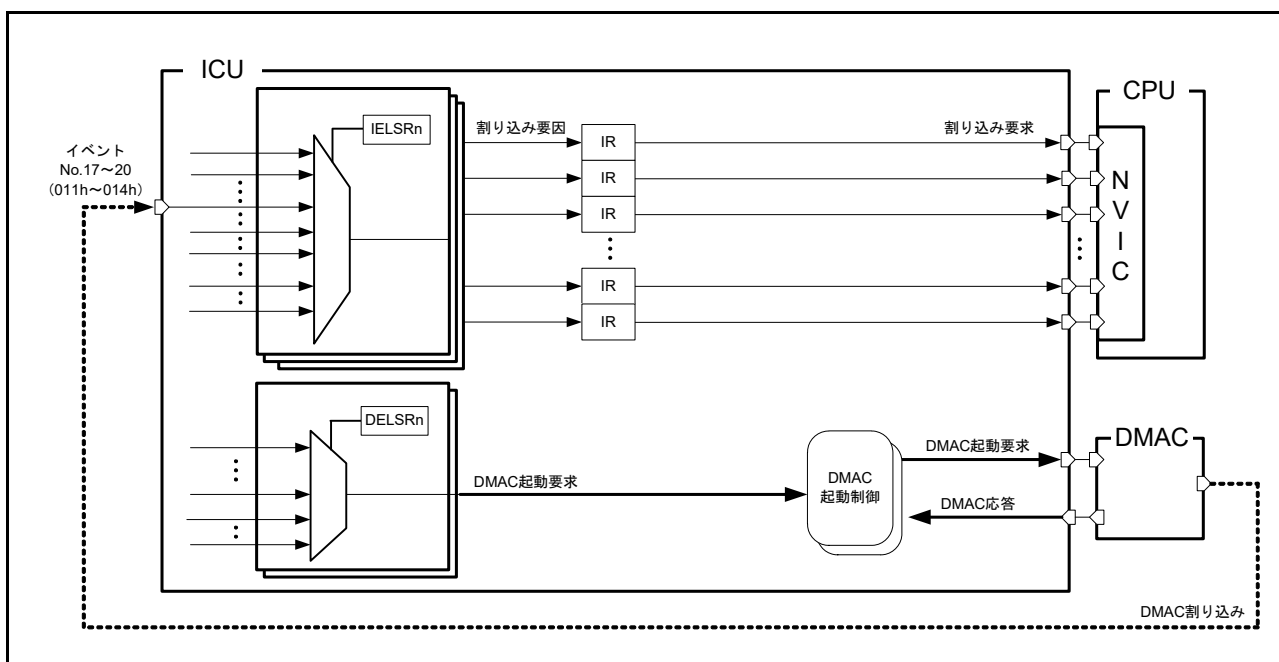
図 13.3 DMAC 要求トリガと割り込み経路
