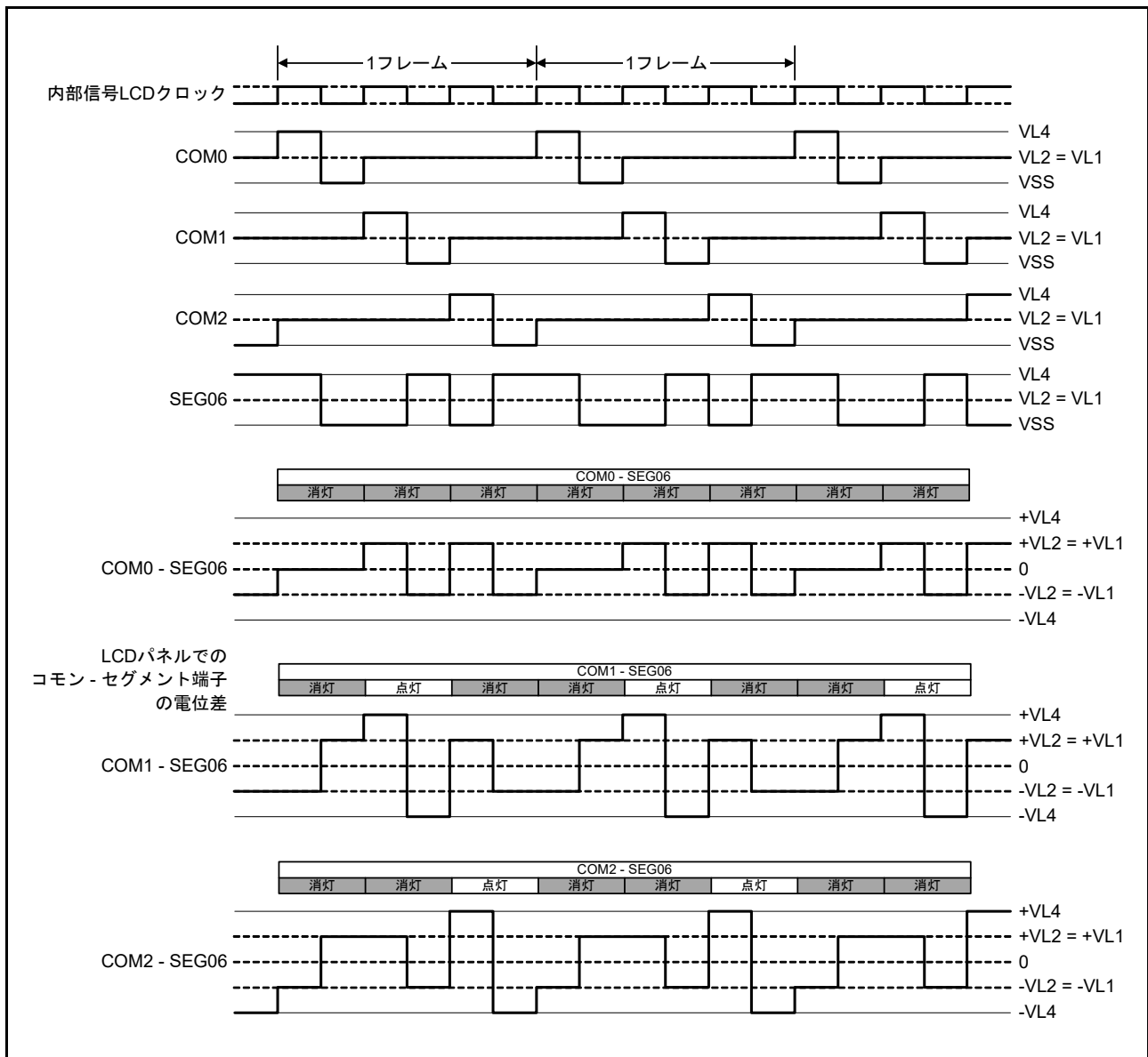
図 45.26 1/2 バイアス法を用いた SEG06 と各コモン信号との間の 3 時分割 LCD 駆動波形例
