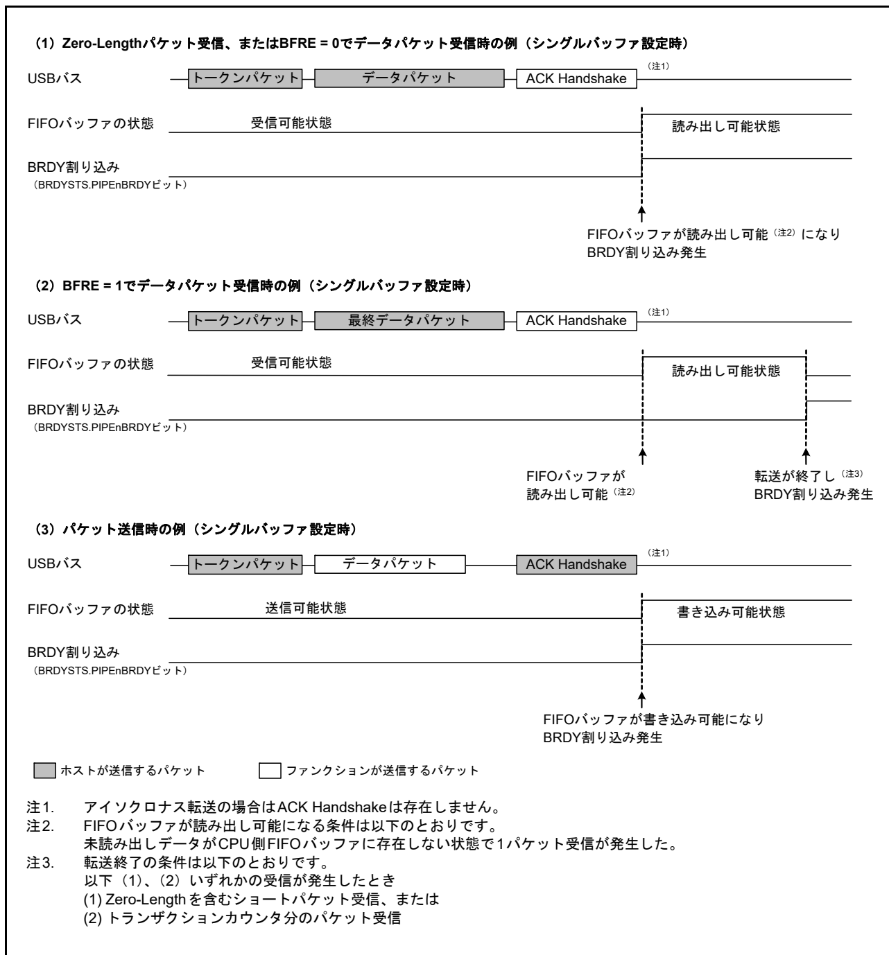
図 27.12 BRDY 割り込みの発生タイミング
