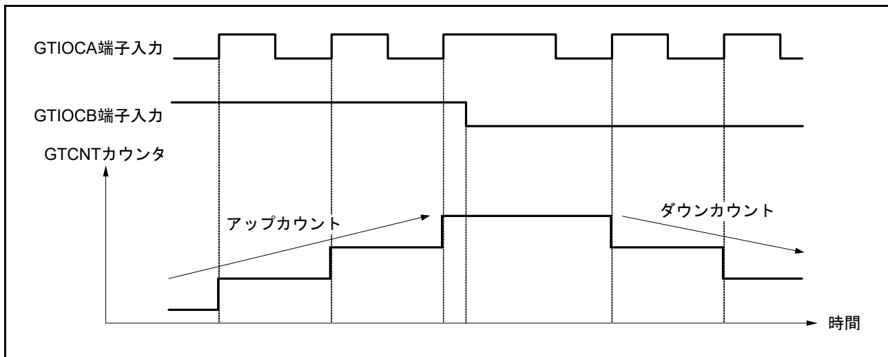
図 22.69 位相計数モード2 動作例 (B)
