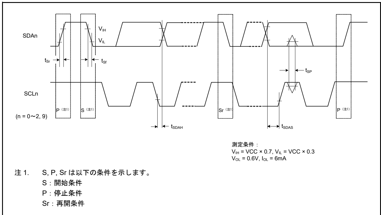
図 47.51 SCI 簡易 IIC モードタイミング
