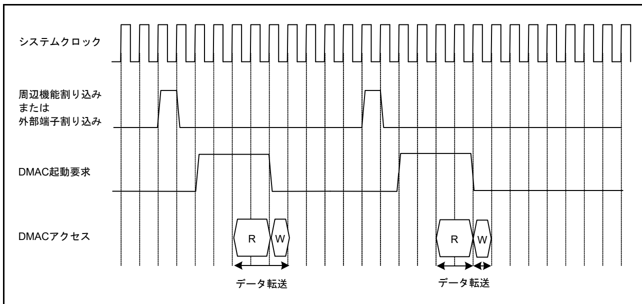
図 16.10 DMAC 動作タイミング例 1 (ノーマル転送モードまたはリピート転送モードでの周辺モジュール/外部割り込み入力端子からの割り込みによる DMA 起動)
