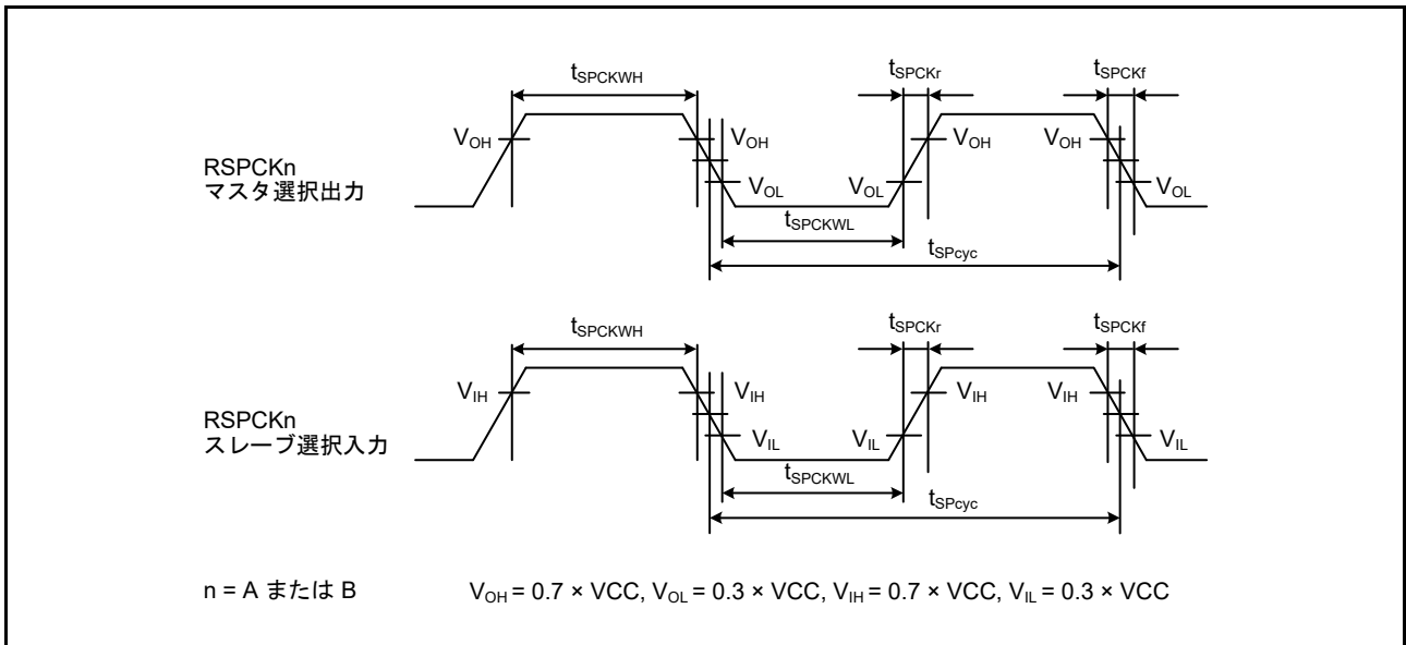
図 47.52 SPI クロックタイミング
