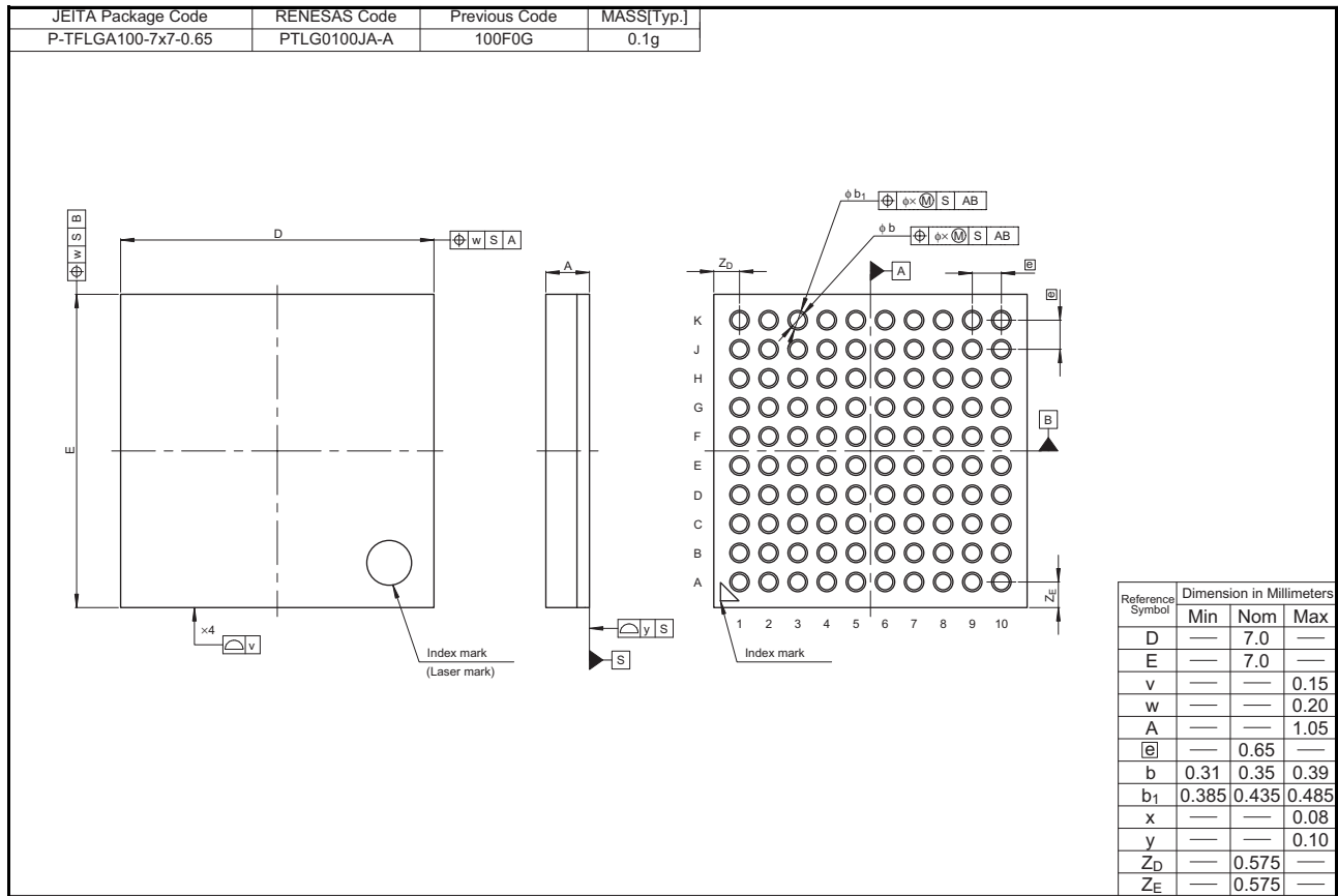
図 2.1 100-pin LGA
