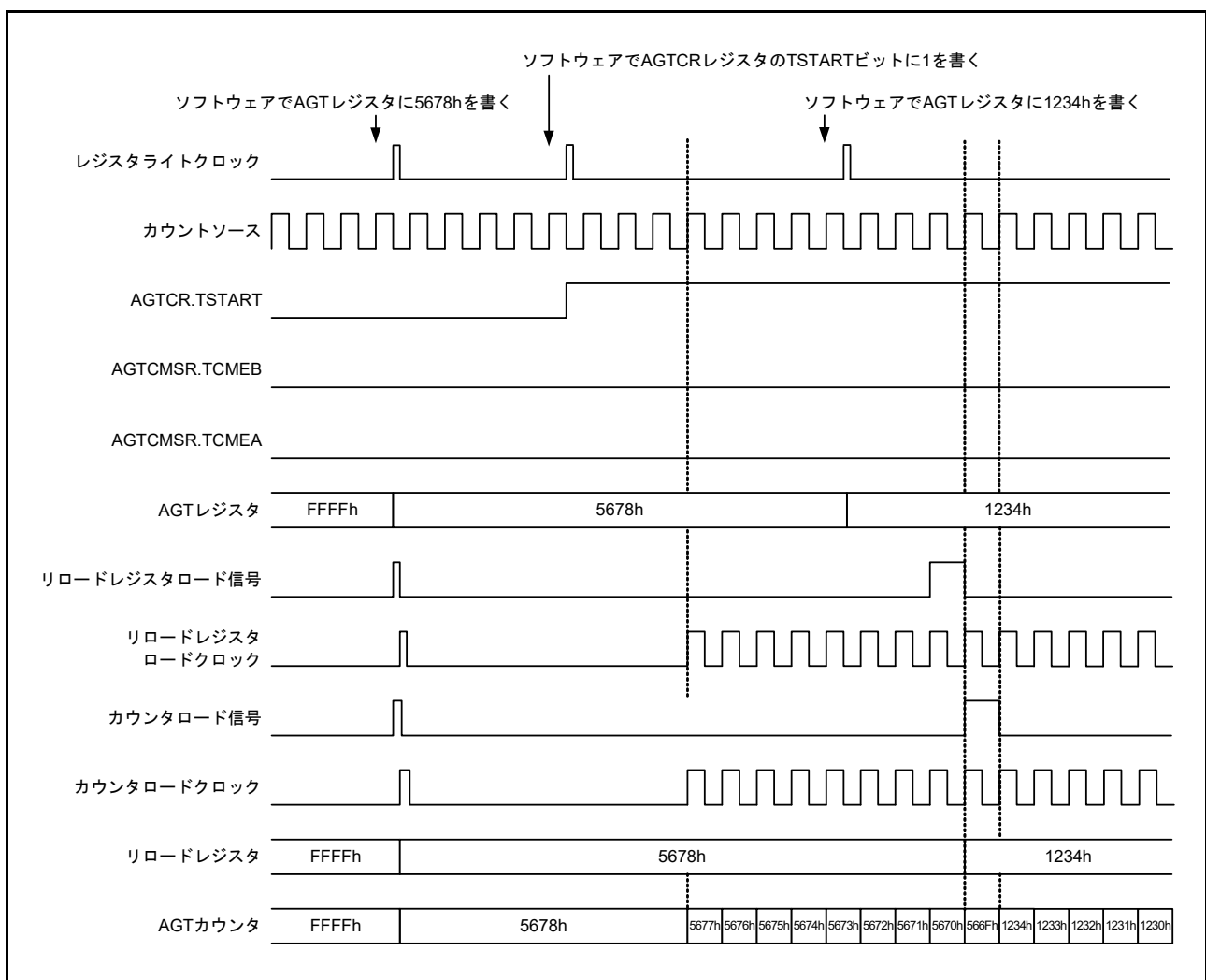
図 23.2 TSTART ビット値および TCMEA または TCMEB ビット値による書き換え動作のタイミング (コンペアマッチ A レジスタまたはコンペアマッチ B レジスタが無効の場合)
