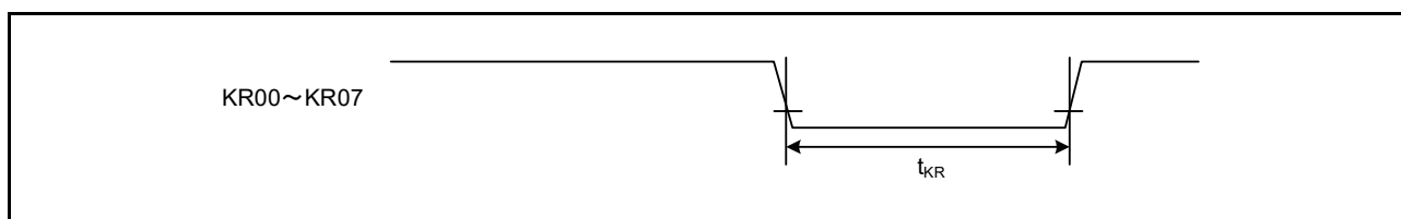
図 47.43 キー割り込み入力タイミング
