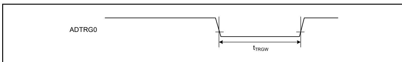
図 47.42 ADC14 トリガ入力タイミング
