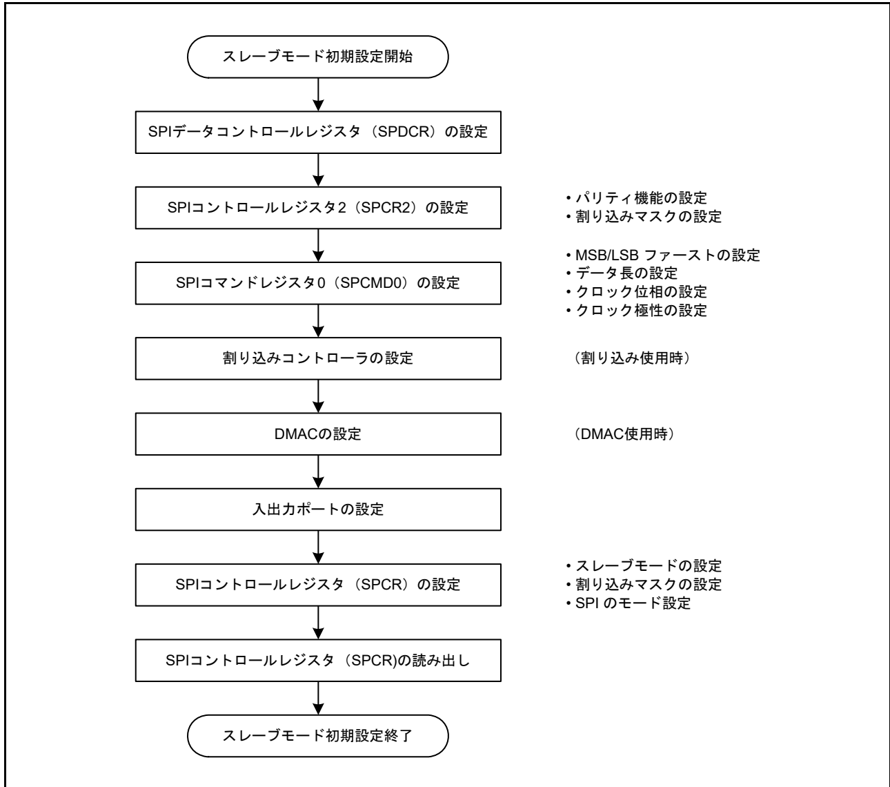
図 31.47 スレーブモード時のクロック同期式動作の初期化フロー例
