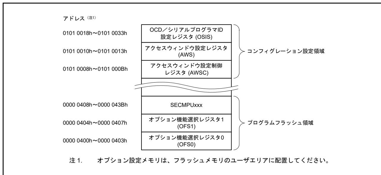
図 6.1 オプション設定メモリの領域
