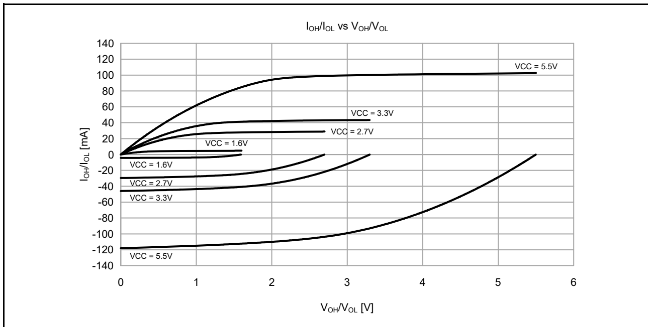
図 47.7 中駆動出力選択時の Ta = 25 °Cでの V OH /V OL および I OH /I OL 電圧特性 (参考データ)
