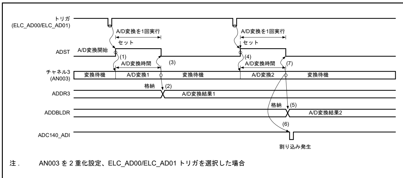
図 35.9 シングルスキャンモードの基本動作例 (ダブルトリガモード選択、AN003を2重化)
