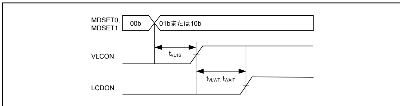
図 47.80 LCD 基準電圧セットアップ時間、昇圧待機時間、容量分割待機時間
