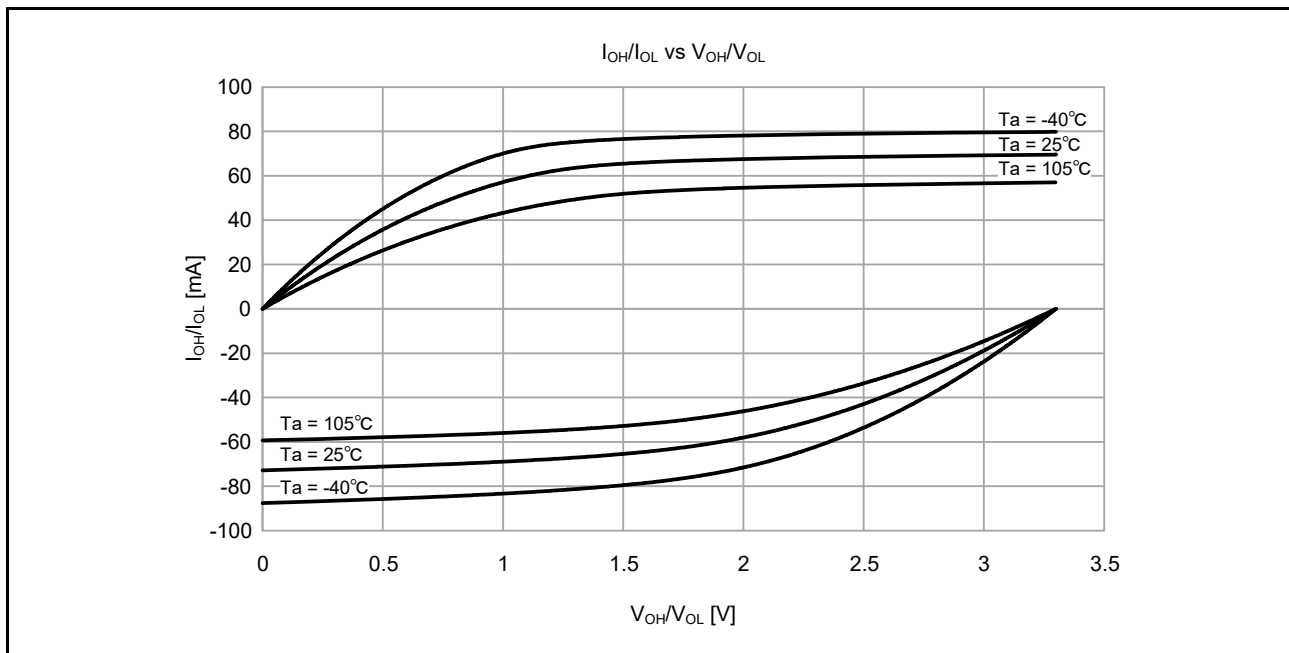
図 47.14 中駆動出力選択時の VCC = 3.3V での V_{OH}/V_{OL} および I_{OH}/I_{OL} 温度特性 (参考データ)
