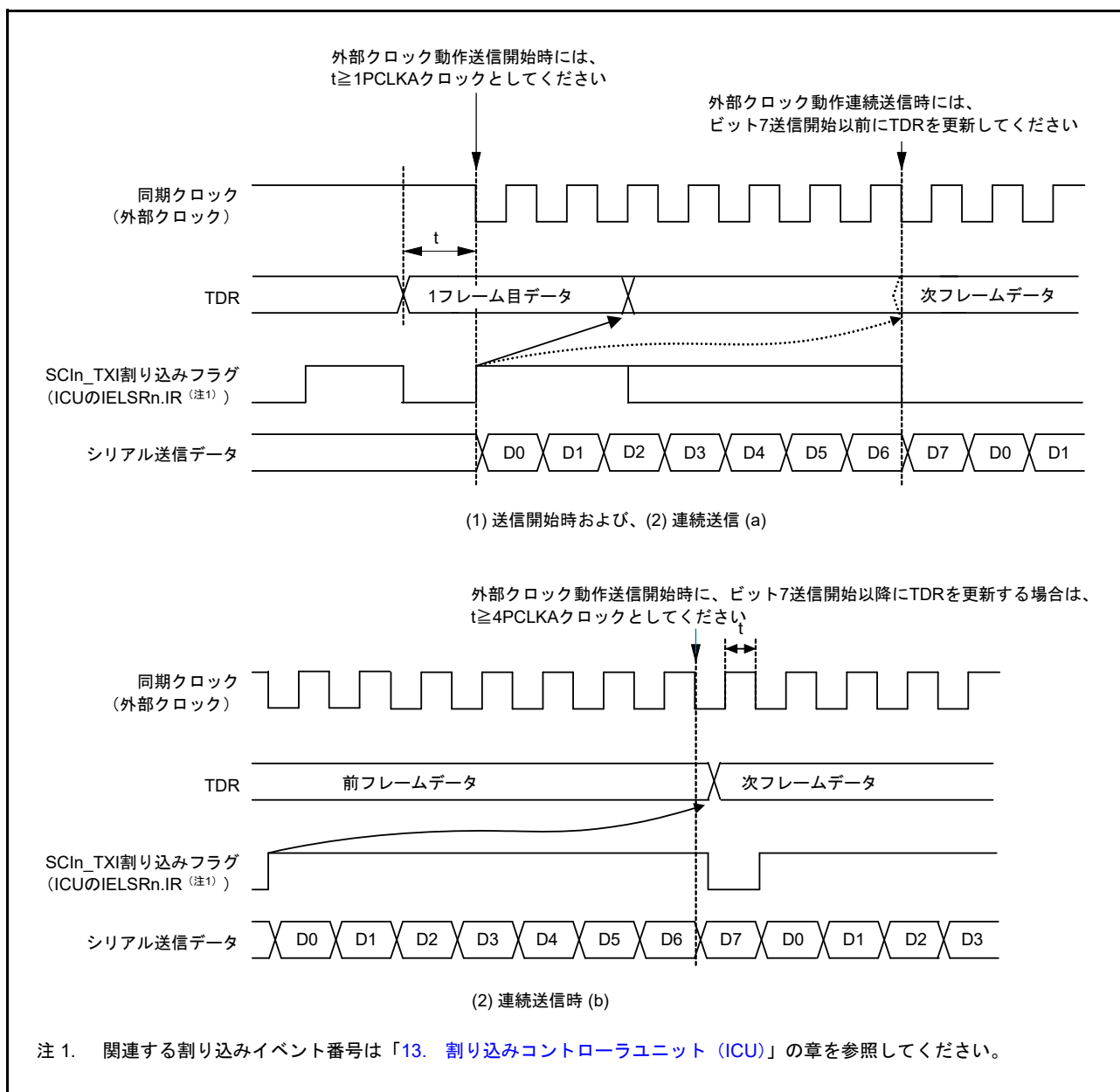
図 28.78 クロック同期送信時の外部クロック使用に関する制限事項
