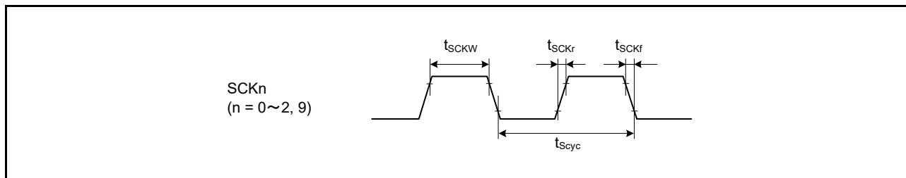
図 47.44 SCK クロック入力タイミング
