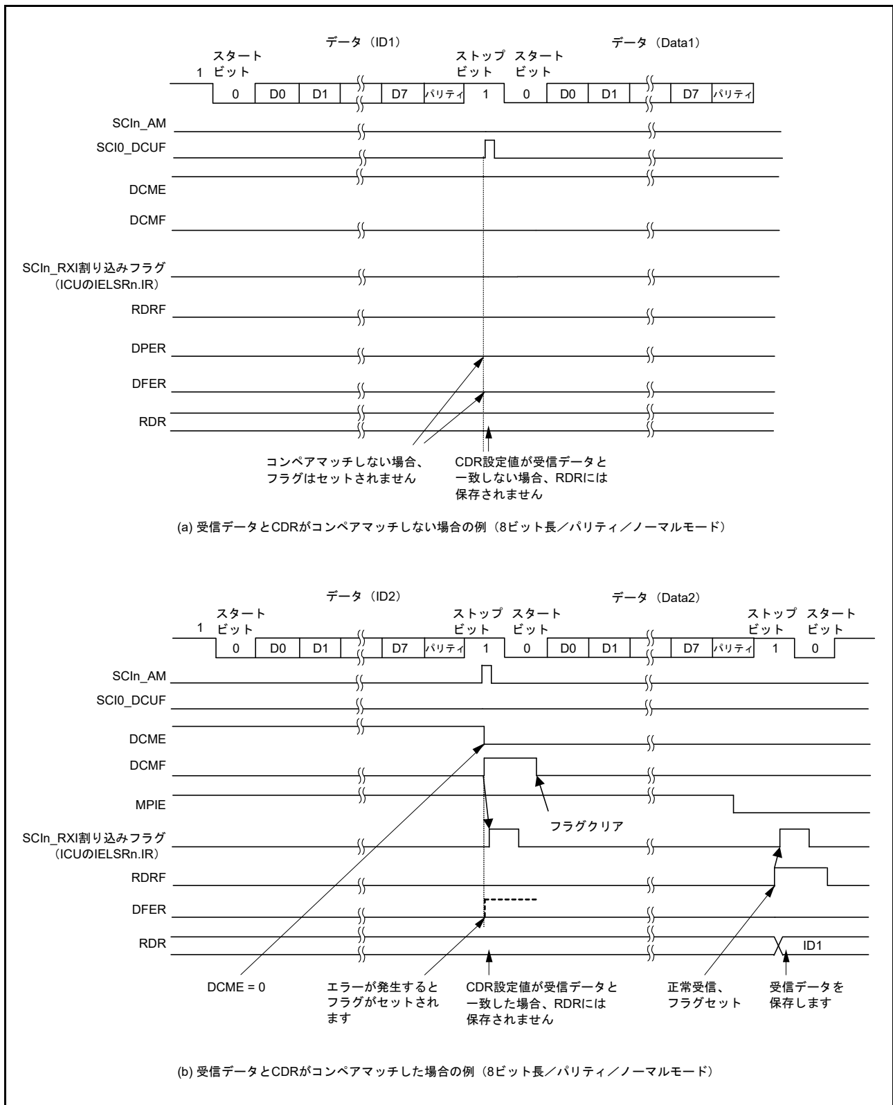
図 28.5 アドレス一致検出の例 (1) (通常モード)
