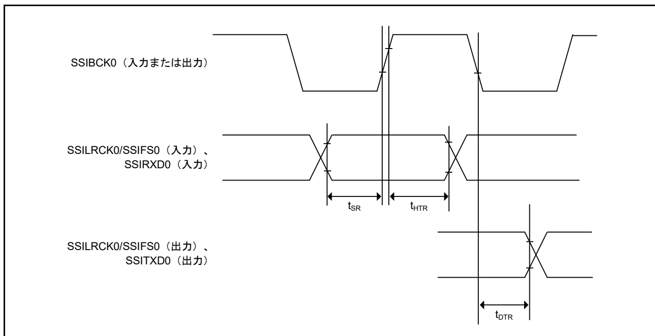
図 47.61 SSIE データ送受信タイミング (SSICR.BCKP = 0)
