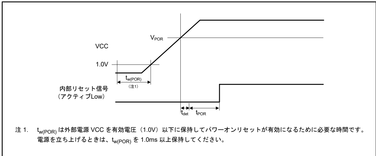
図 47.73 パワーオンリセットタイミング
