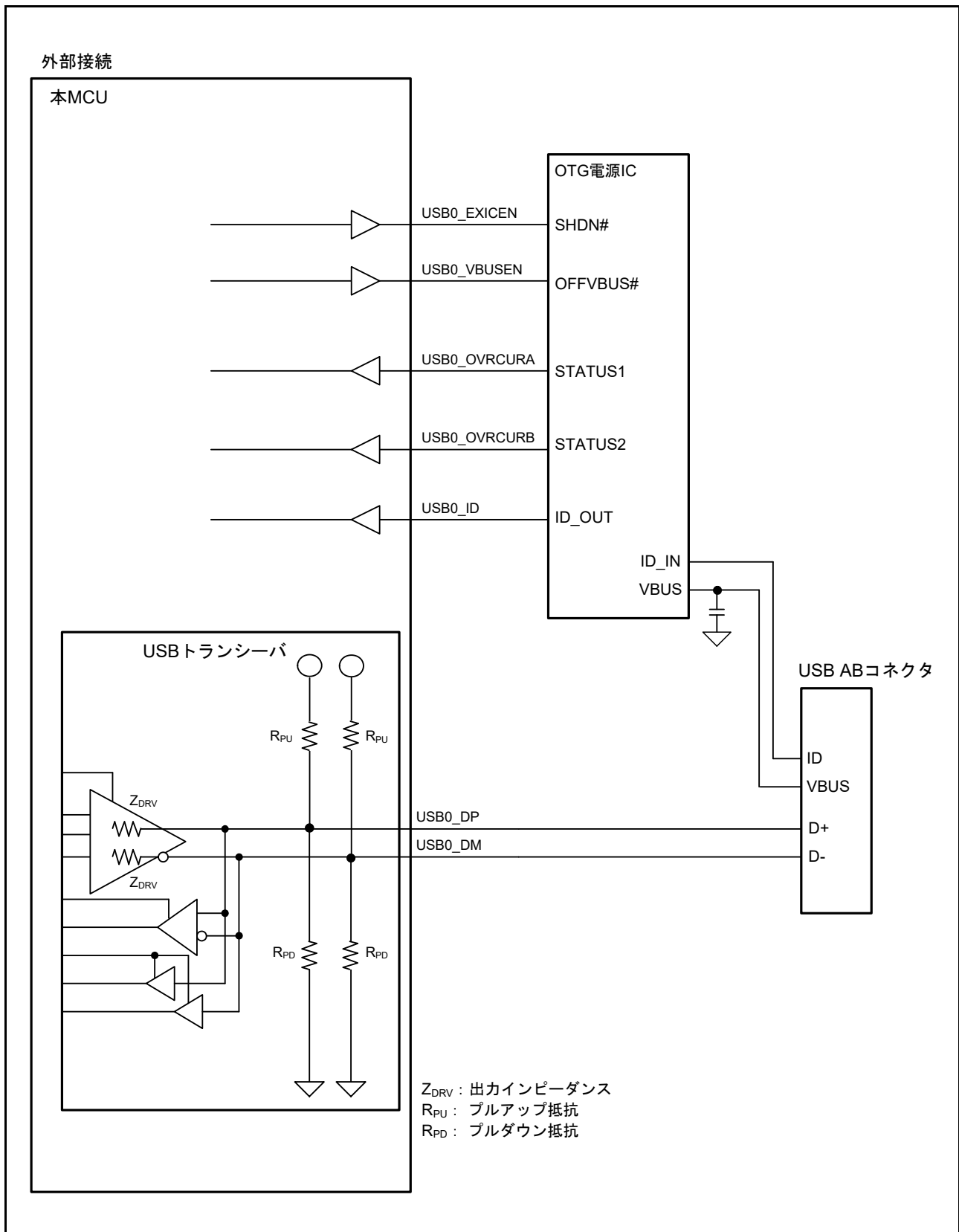
図 27.5 セルフパワー状態での OTG 接続例
