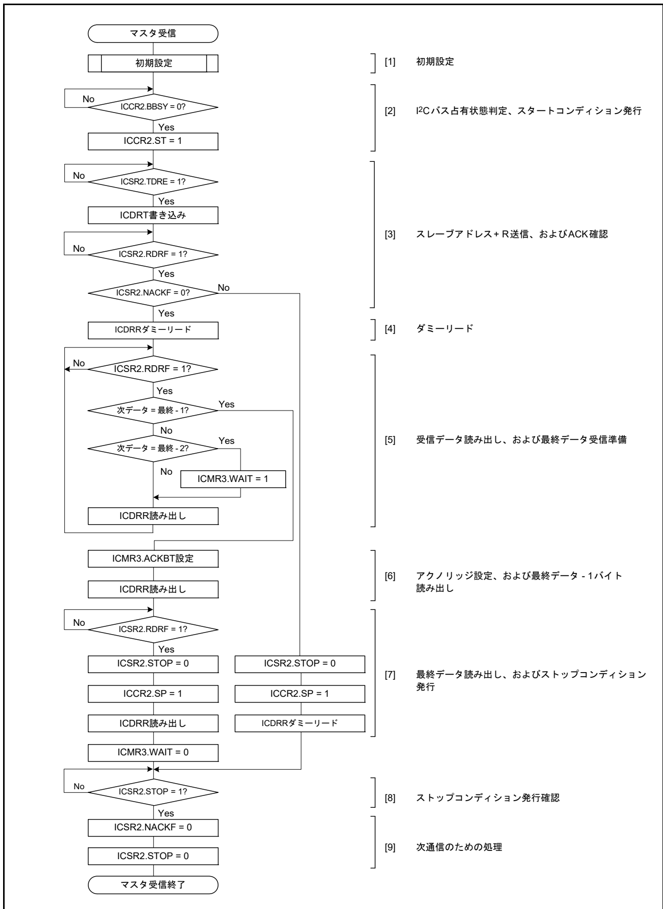
図 29.11 マスタ受信の例 (7ビットアドレスフォーマット、3バイト以上受信時)
