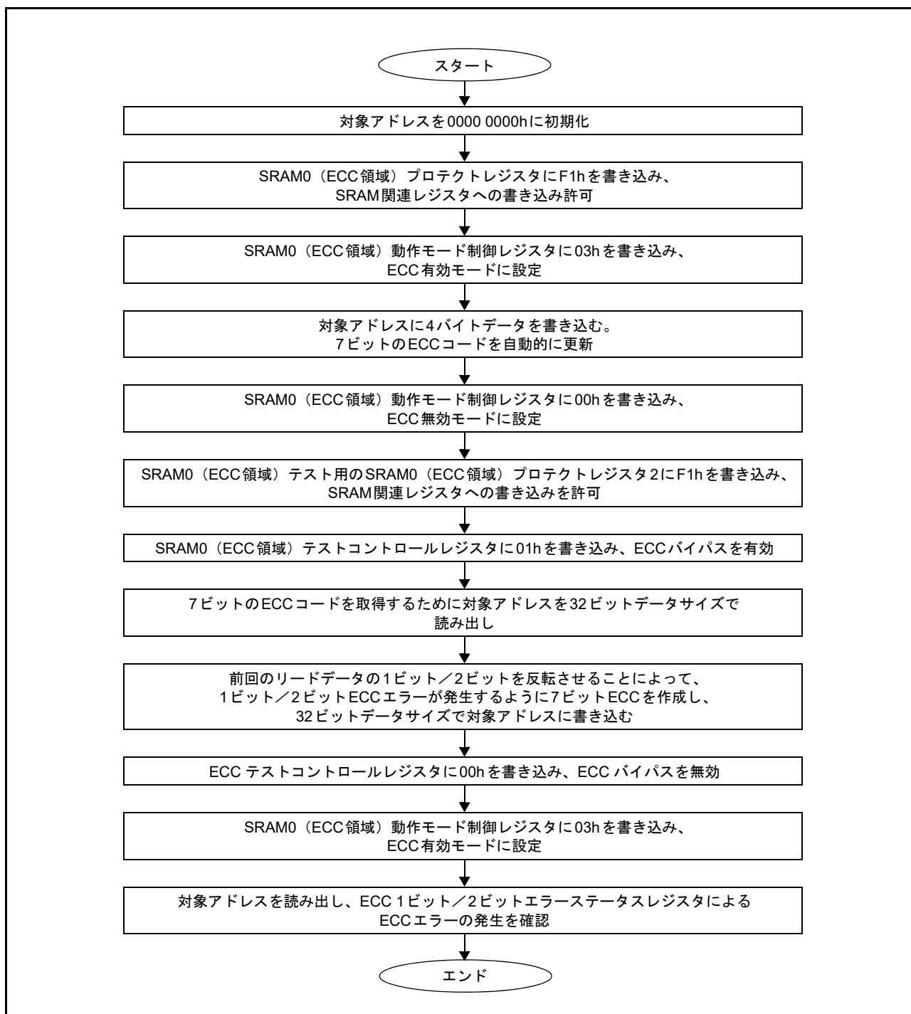
図 43.1 ECC デコーダのテスト方法
