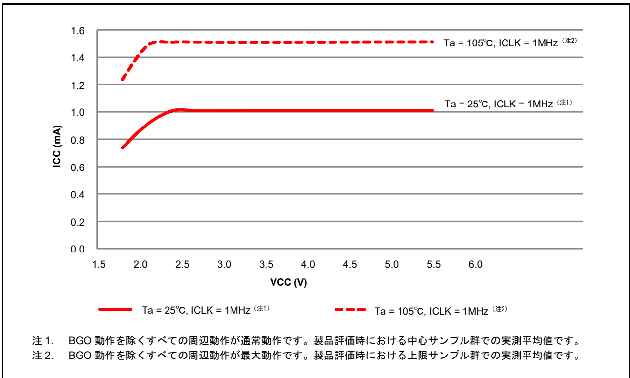
図 47.19 Low-speed モードにおける電圧依存性 (参考データ)
