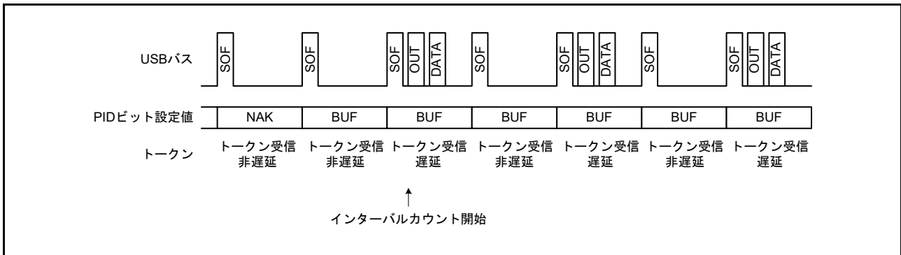
図 27.20 フレームとトークン受信待機の関係 (IITV ≠ 0 の場合)
