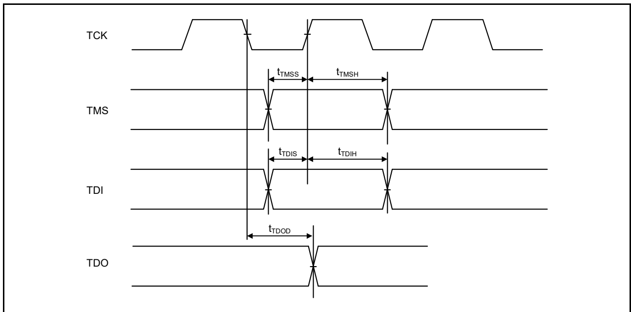
図 47.85 JTAG 入出力タイミング
