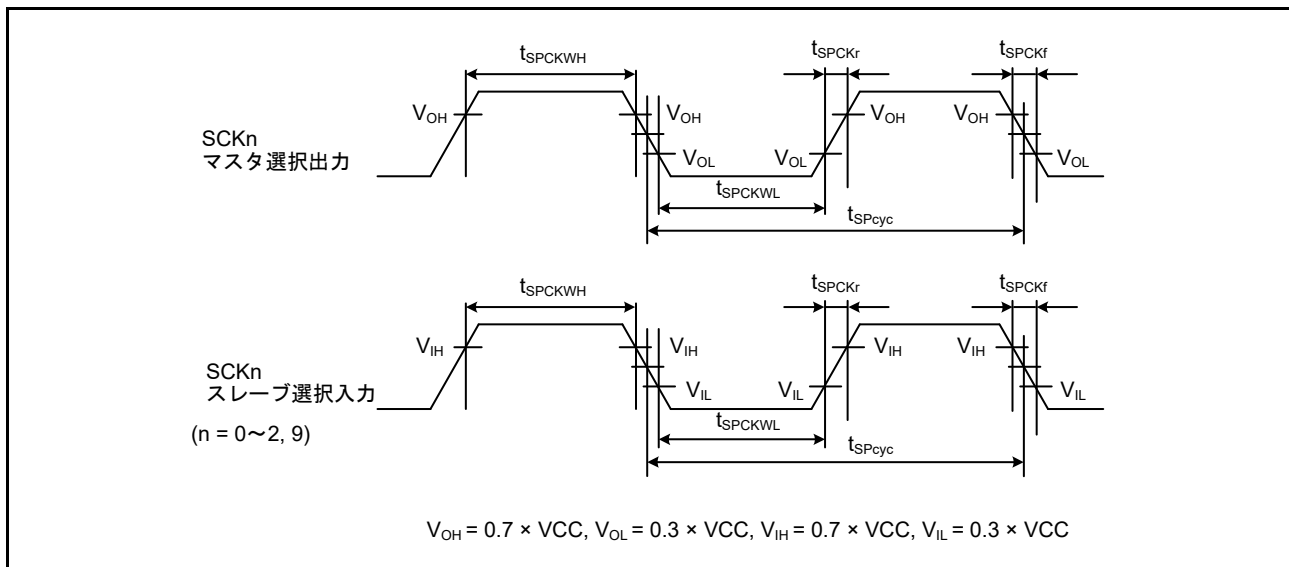
図 47.46 SCI 簡易 SPI モードクロックタイミング
