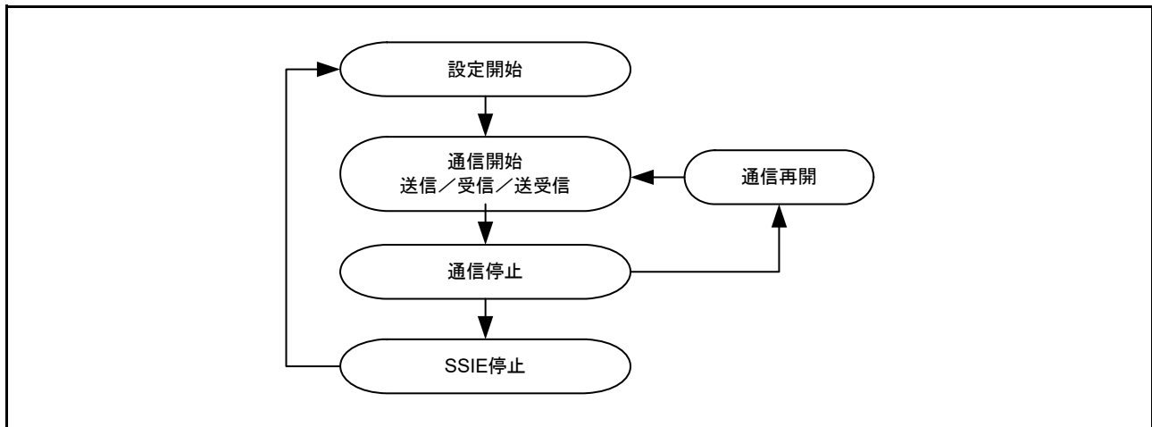
図 33.48 SSIE 通信動作
