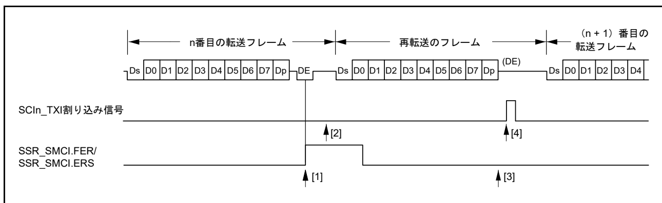
図 28.52 SCI 送信モードでの再転送動作
