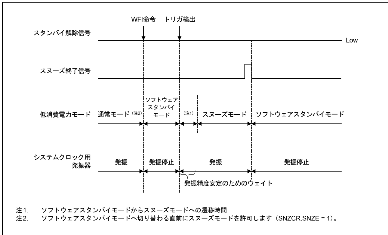
図 10.10 スヌーズモード時に割り込み要求信号が発生しない場合
