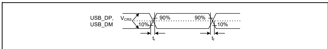
図 47.65 USB_DP および USB_DM 出力タイミング
