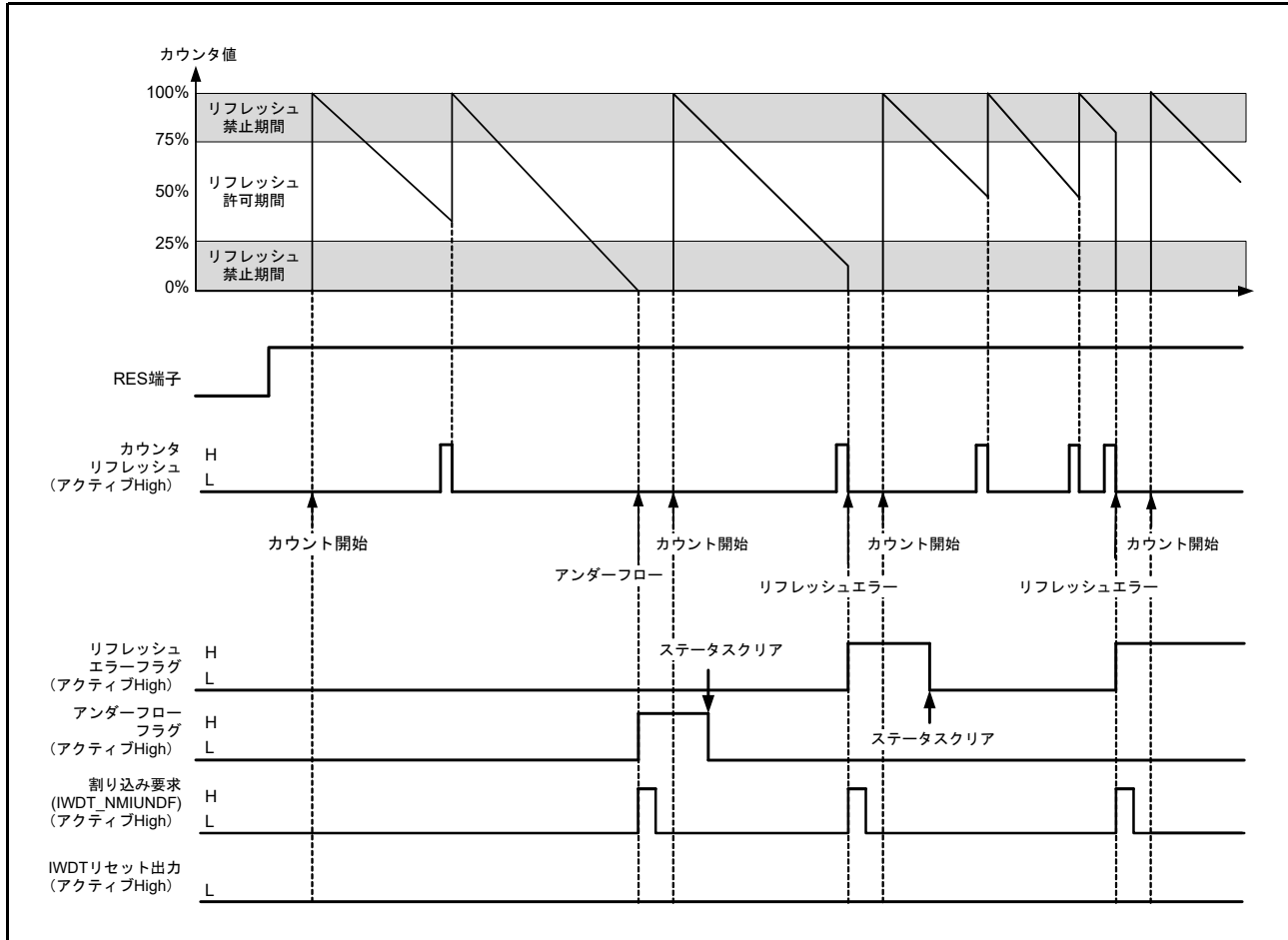
図 26.3 オートスタートモードでの動作例
