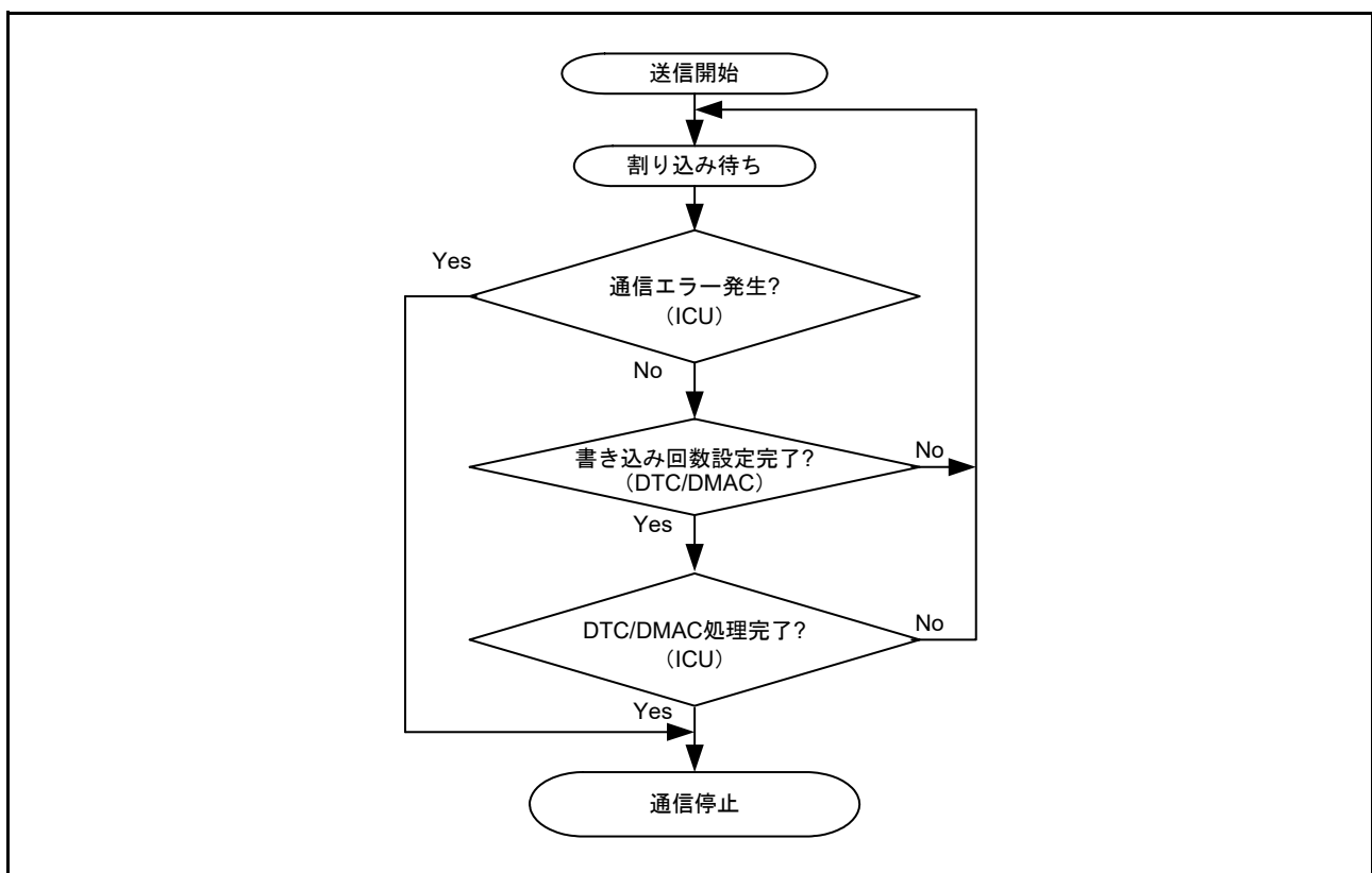
図 33.50 送信手順
