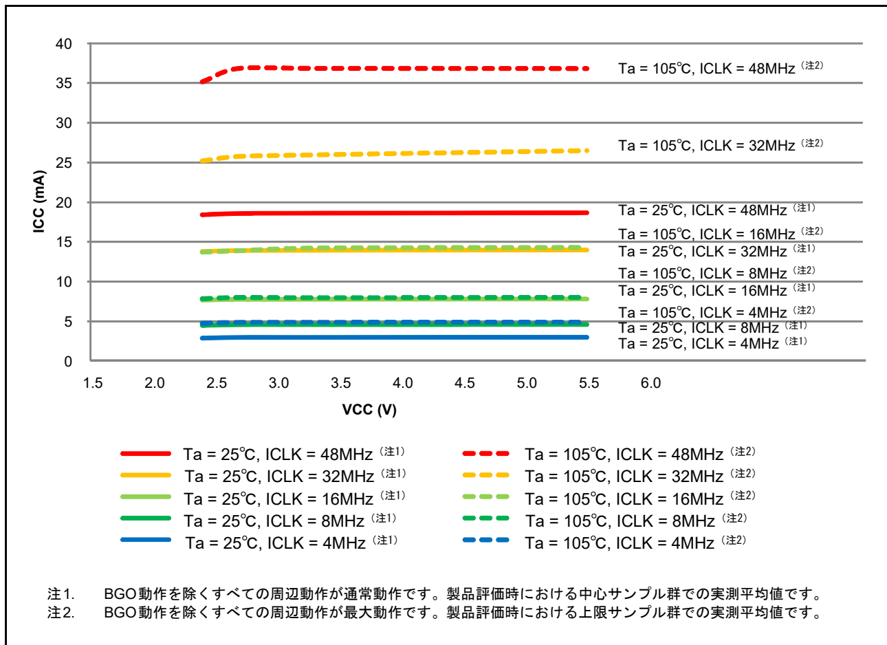
図 47.17 High-speed 動作モードにおける電圧依存性 (参考データ)
