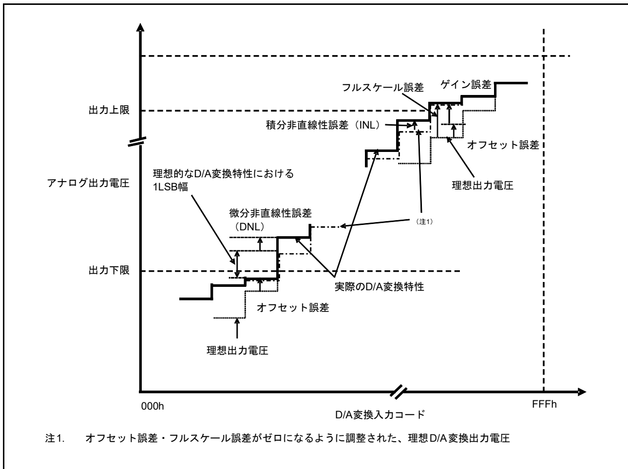
図 47.70 D/A コンバータ特性用語の解説図
