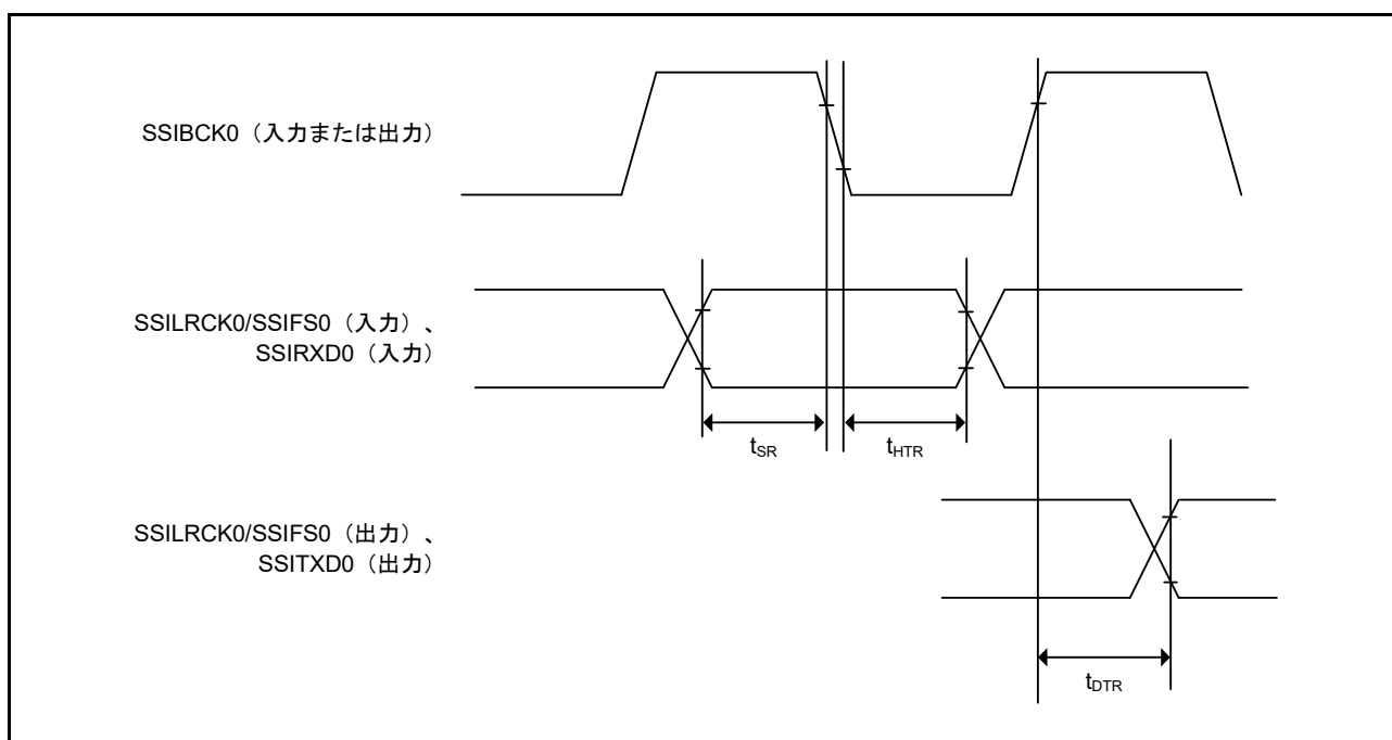
図 47.62 SSIE データ送受信タイミング (SSICR.BCKP = 1)
