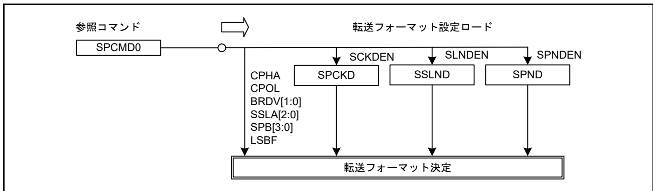
図 31.32 マスタモードでのシリアル転送方式の決定方法
