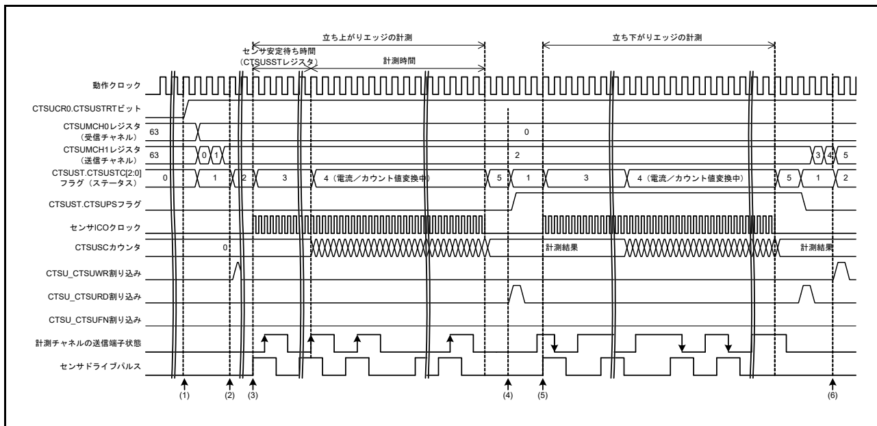
図 41.17 相互容量フルスキャンモードのタイミング (計測開始条件がソフトウェアトリガの場合)
