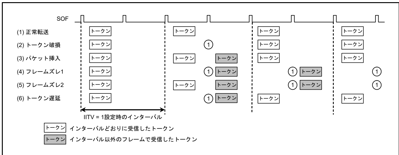
図 27.23 IITV = 1 の場合のインターバルエラー発生例
