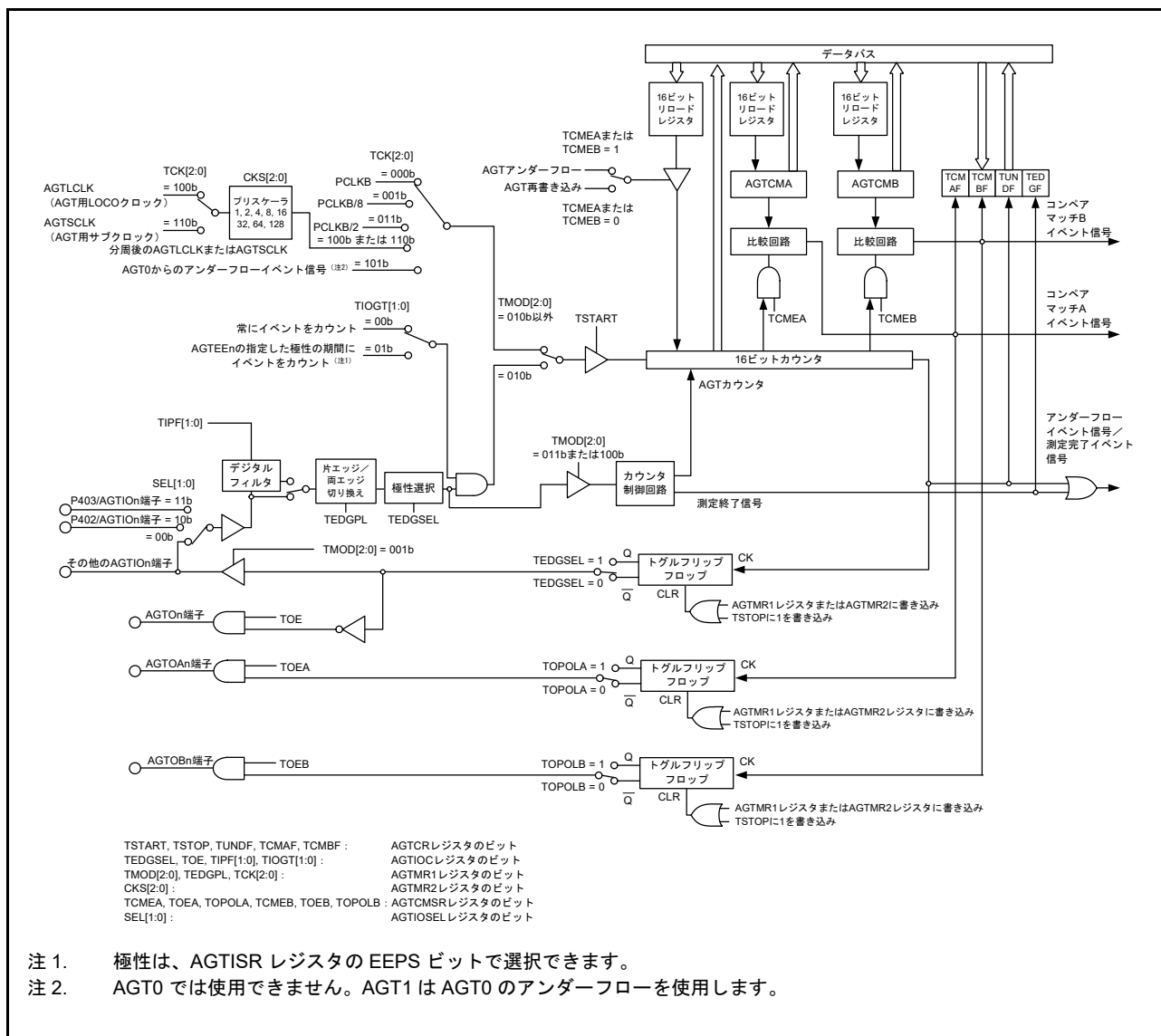
図 23.1 AGT のブロック図
