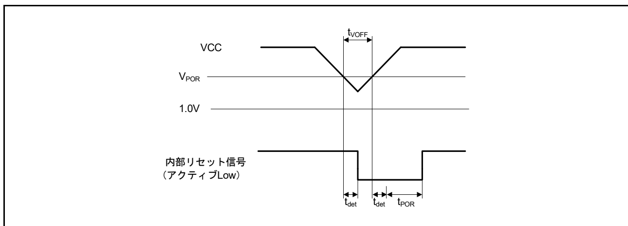
図 47.72 電圧検出リセットタイミング
