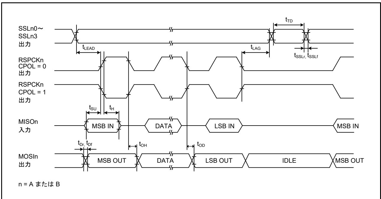
図 47.53 SPI タイミング (マスタ、CPHA = 0) (ビットレート : PCLKA を 2 分周以外に設定)
