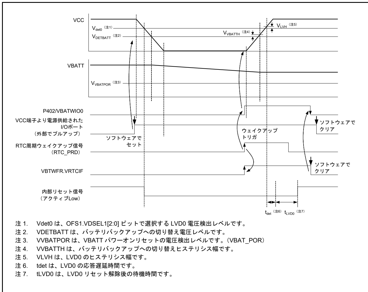
図 11.6 VBAT ウェイクアップ機能のタイミング図
