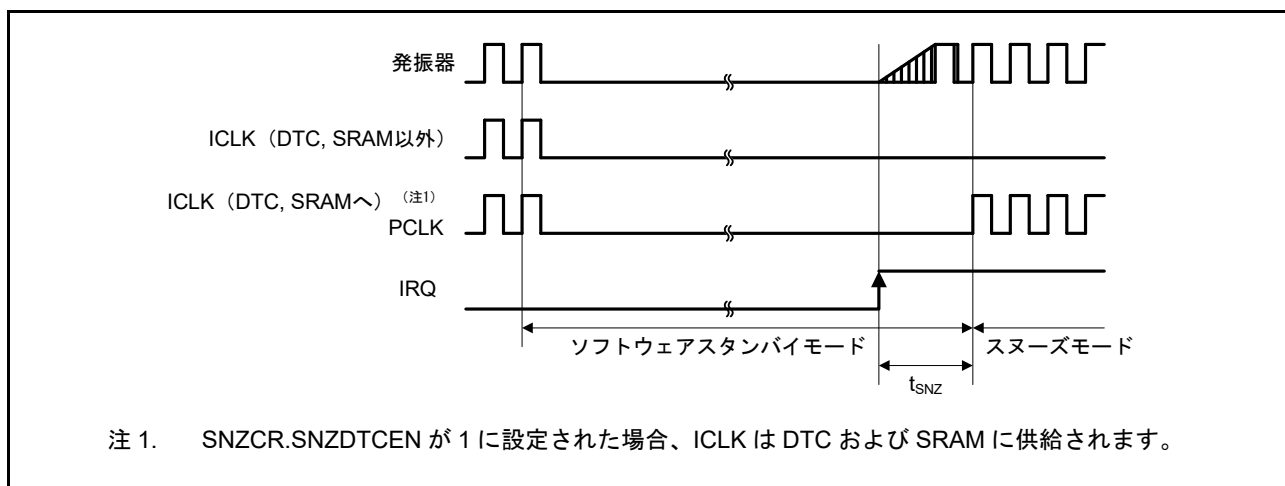
図 47.35 ソフトウェアスタンバイモードからスヌーズモードへの復帰タイミング
