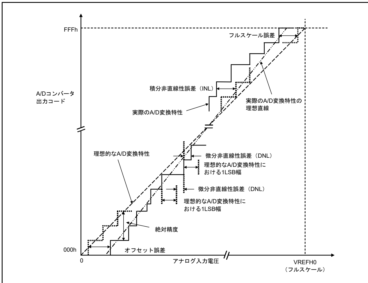
図 47.69 14 ビット A/D コンバータ特性用語の解説図
