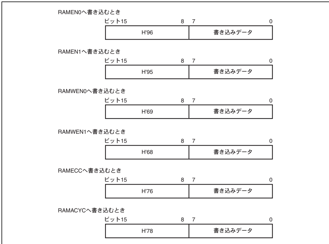
図 28.3 RAMEN0、1、RAMWEN0、1、RAMECC、および RAMACYC レジスタへの書き込み
