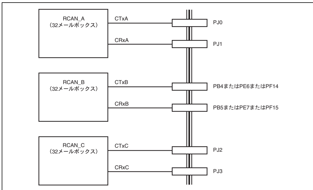
図 18.31 RCAN_A、B、C を個別のチャンネルとして使用する際の接続例
