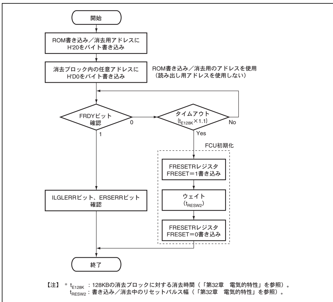
図 25.19 ROM 消去方法
