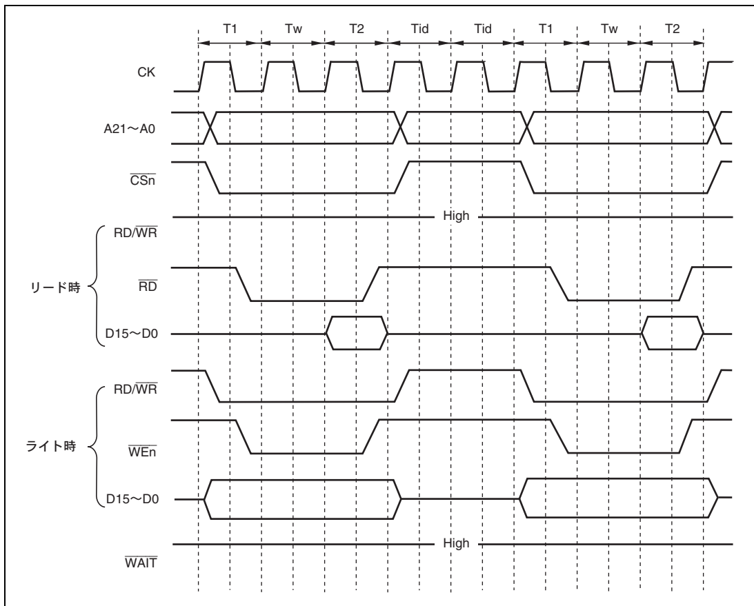
図 10.6 周辺クロック 2 通倍設定時の連続アクセス バス幅 16 ビット、ロングワードアクセス (アクセスウェイト 1、サイクル間ウェイト 2)
