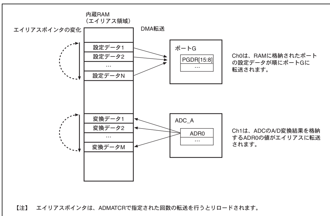
図 12.3 転送の概要 (ATU-III (タイマ G) 用チャンネル、ADC 用チャンネル)
