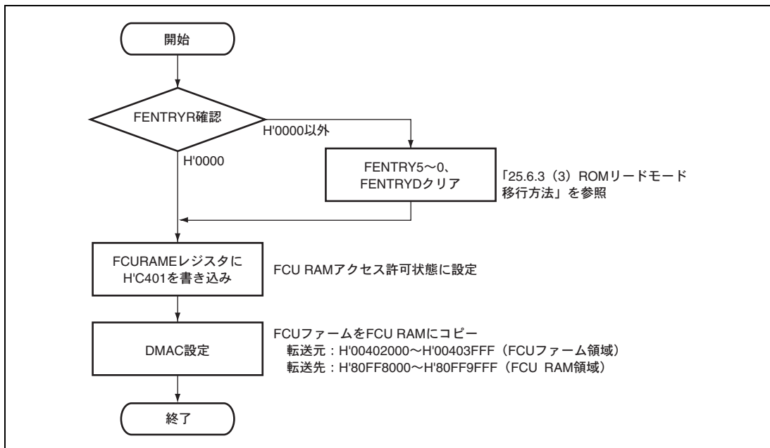
図 25.14 FCU RAM へのファームウェア転送フロー
