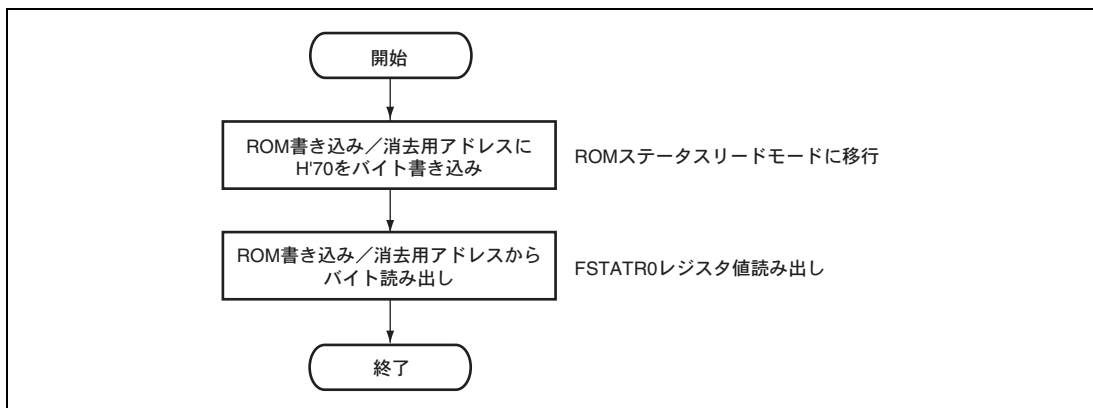
図 25.23 ステータスレジスタ 0 の確認方法
