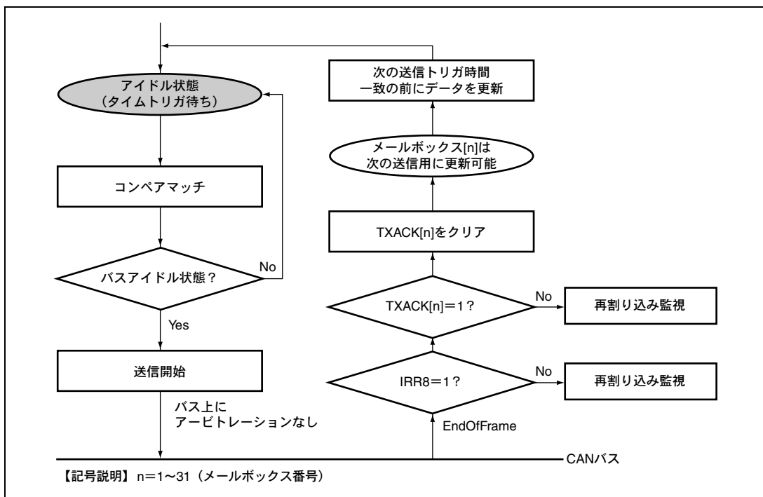
図 18.23 メッセージ送信リクエスト
