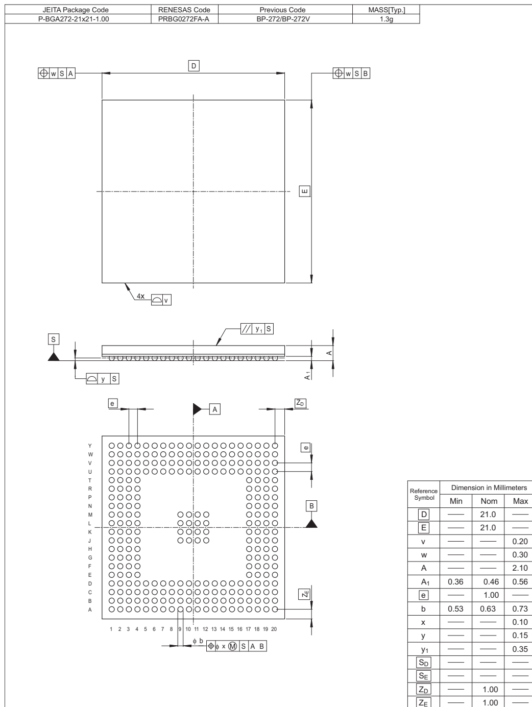
図 C.1 外形寸法図
