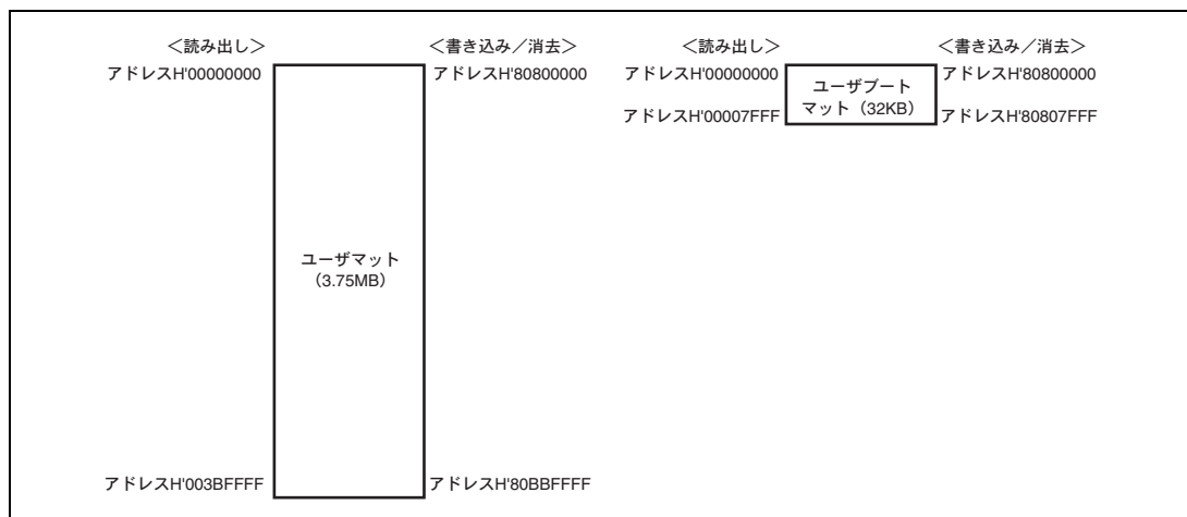
図 25.1 ROM のメモリマット構成
