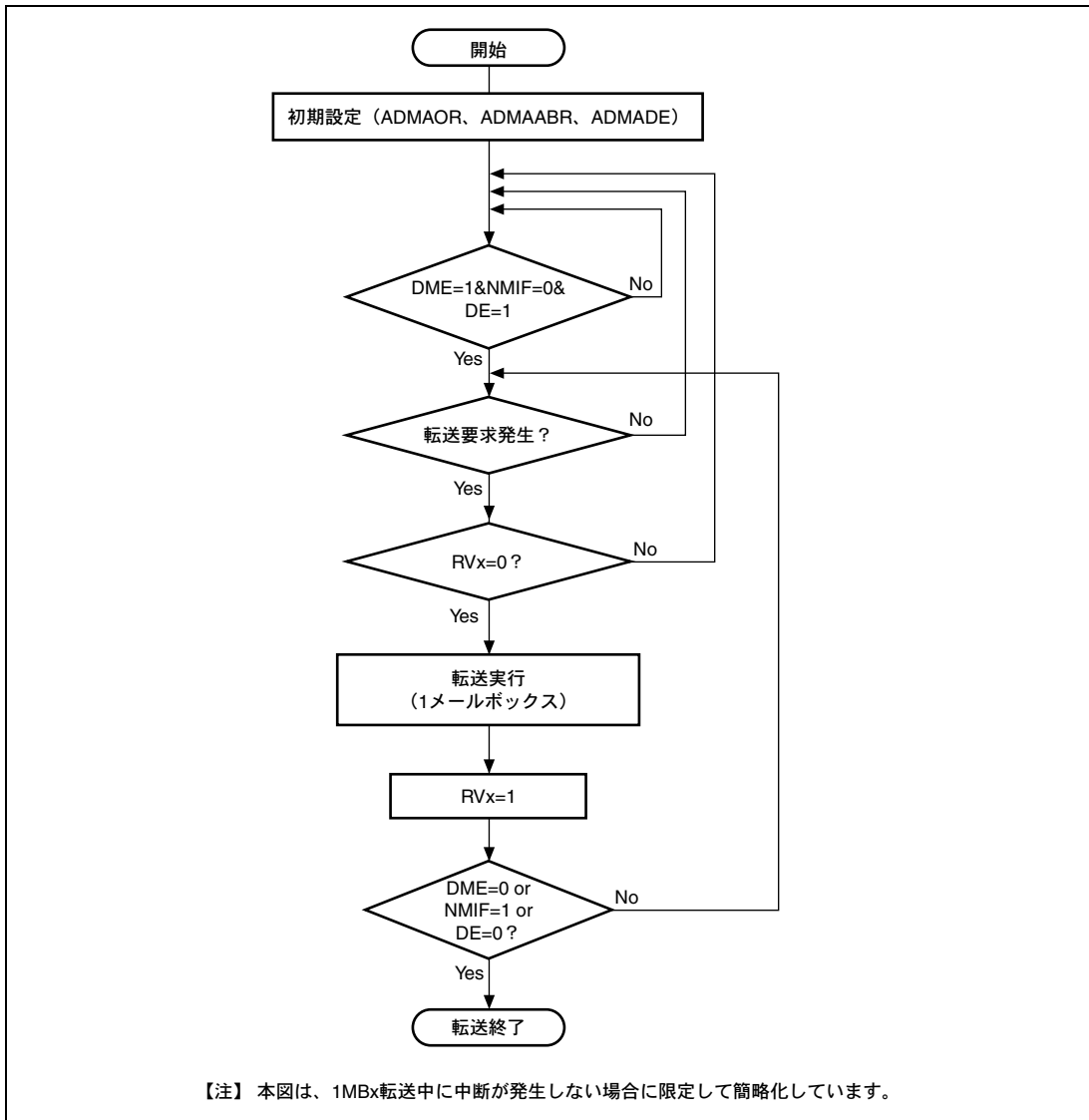
図 12.7 DMA 転送フローチャート (RCAN 用受信用チャンネル)
