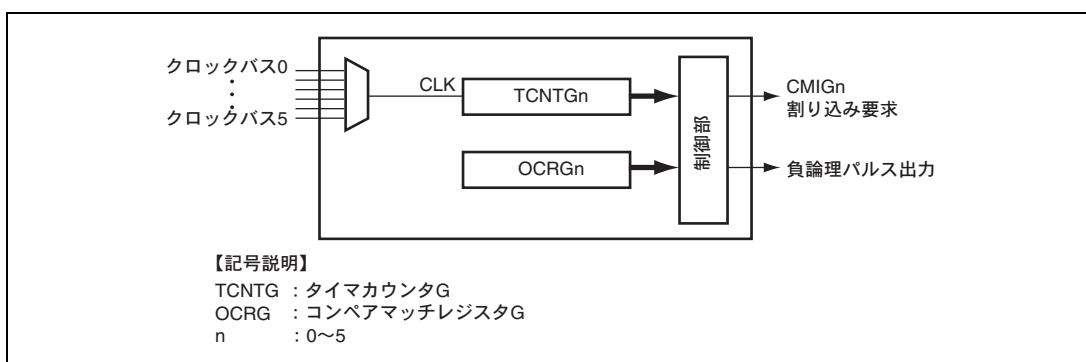
図 13.45 タイマ G のブロック図
