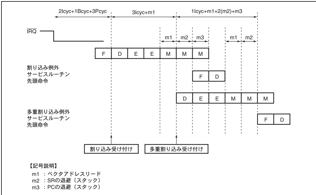
図 8.5 多重割り込み時のパイプライン動作例 (レジスタバンクなし)
