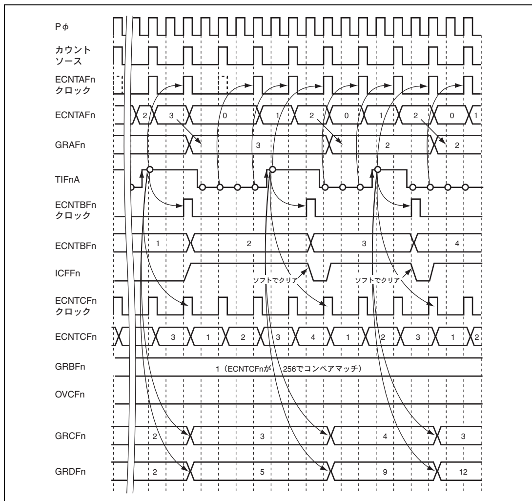
図 13.42 回転速度/パルス計測の動作例
