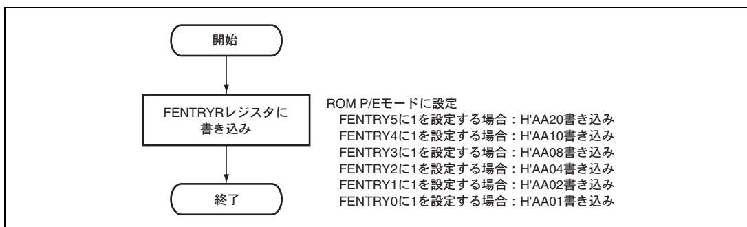
図 25.15 ROM P/E モード移行フロー
