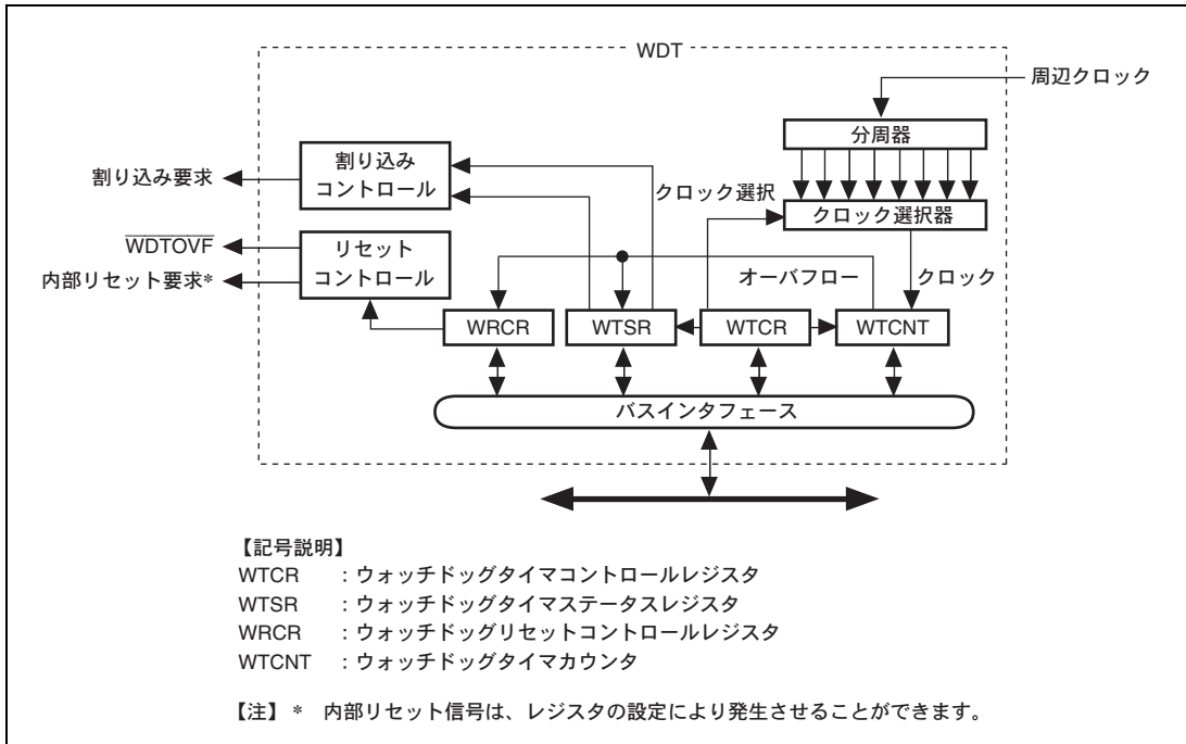
図 14.1 WDT のブロック図
