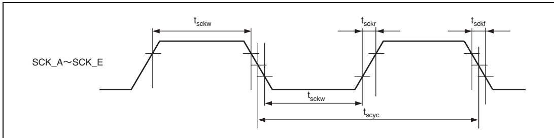
図 32.18 SCK 入力タイミング
