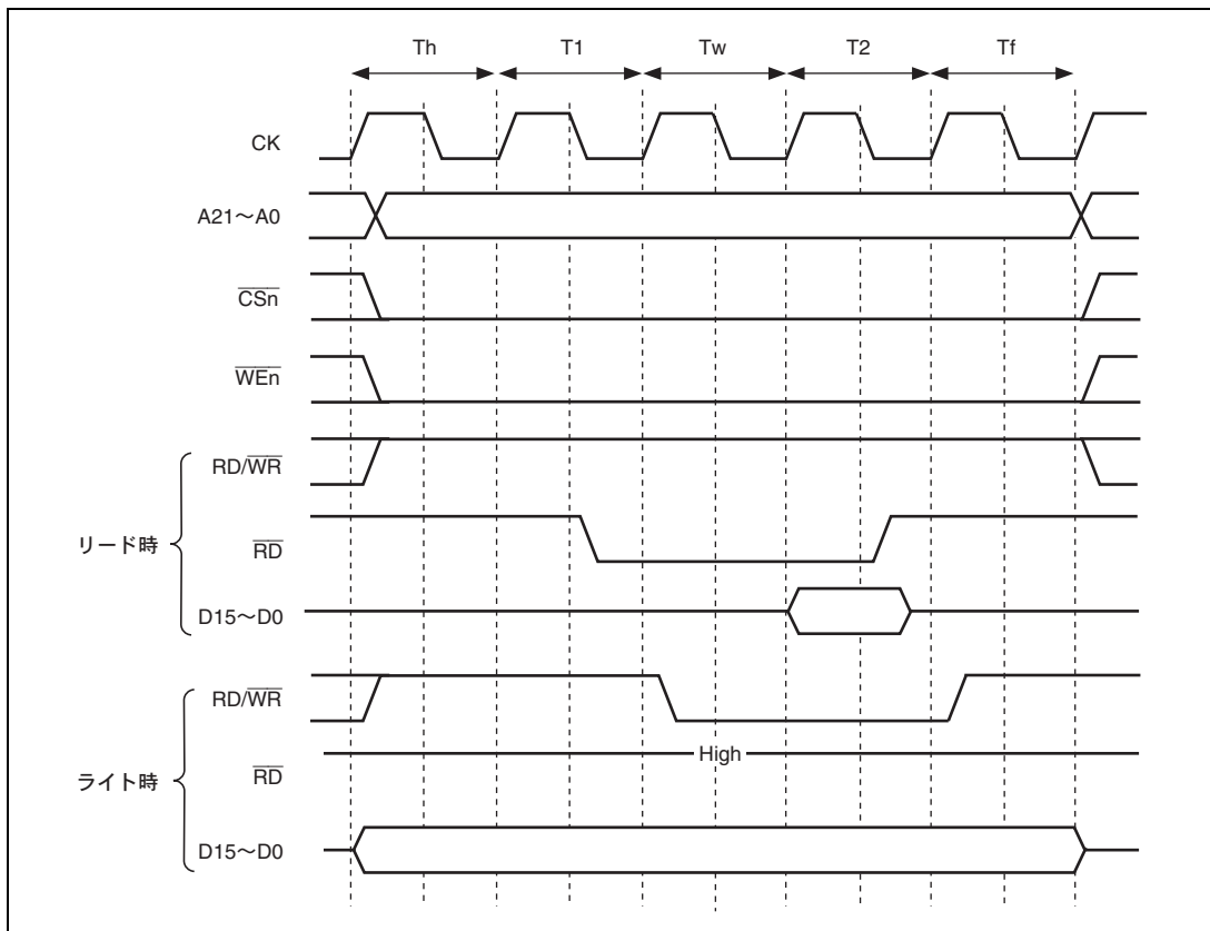
図 10.14 BAS=1、バイト選択付き SRAM ウェイトタイミング (SW[1:0]=01、WR[3:0]=0001、HW[1:0]=01)
