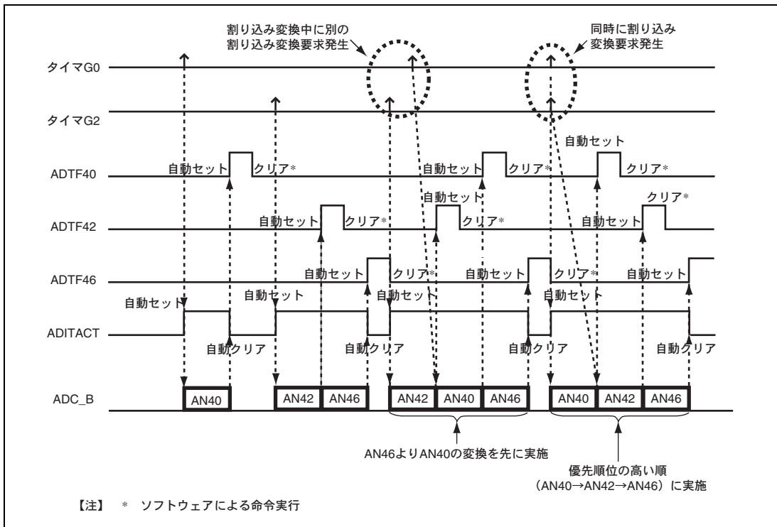
図 19.6 割り込み変換の動作例
