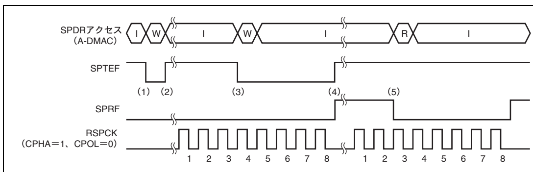
図 17.14 SPTEF、SPRF ビットの動作例
