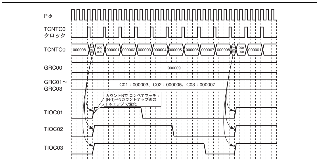
図 13.26 PWM モードの動作例
