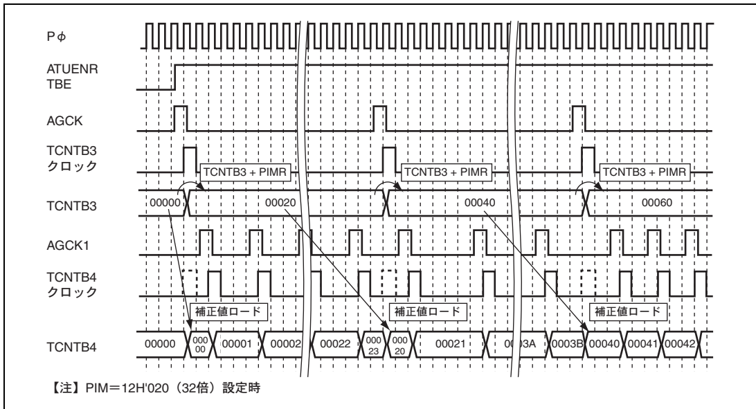
図 13.19 TCNTB3、TCNTB4 の動作
