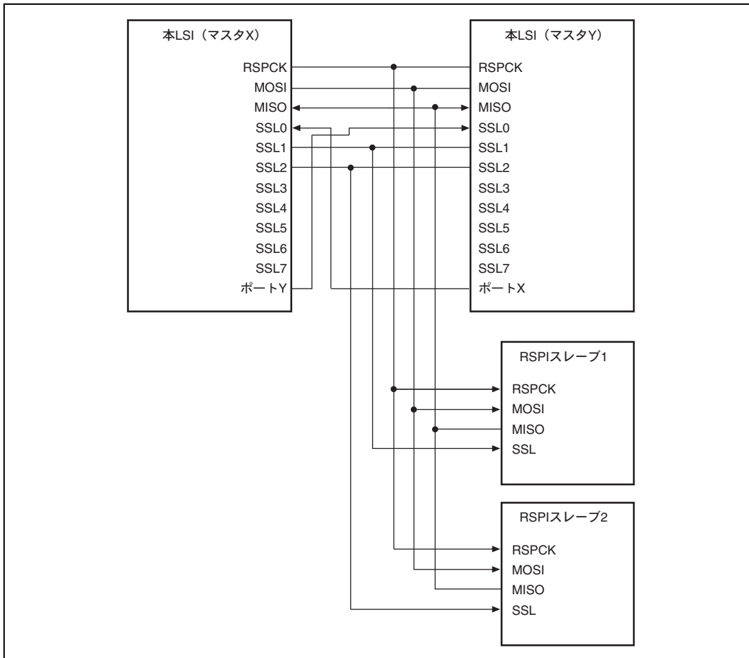
図 17.7 マルチマスタ/マルチスレーブの構成例 (本LSI=マスタ)
