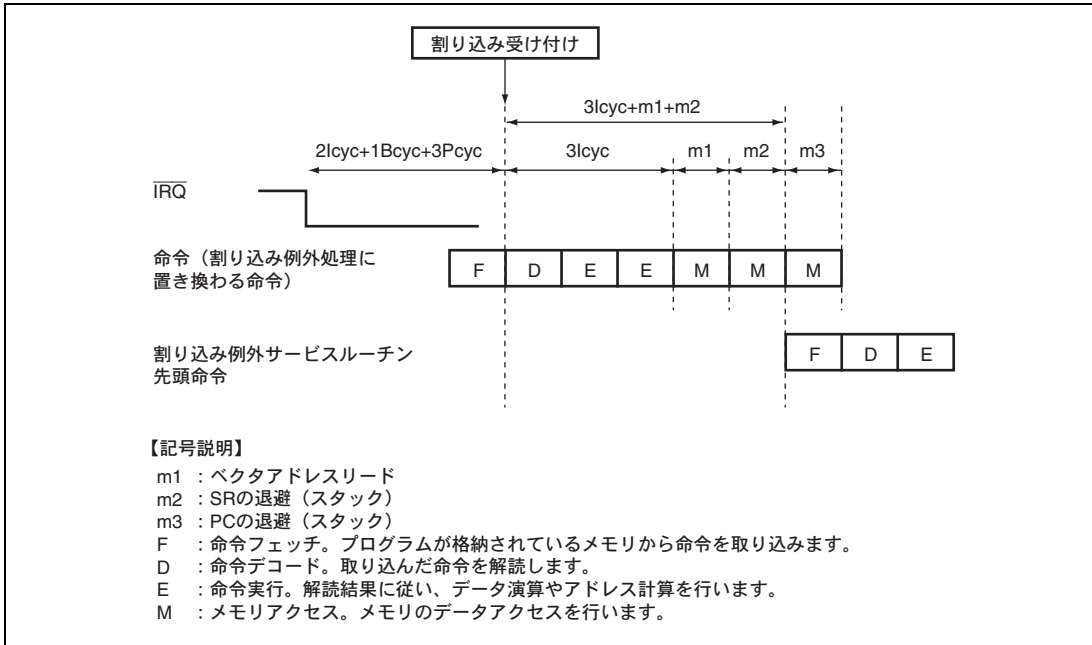
図 8.4 IRQ 割り込みを受け付けるときのパイプライン動作例 (レジスタバンクなし)
