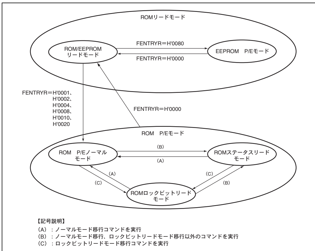
図 25.13 FCU のモード遷移図 (ROM 関連)
