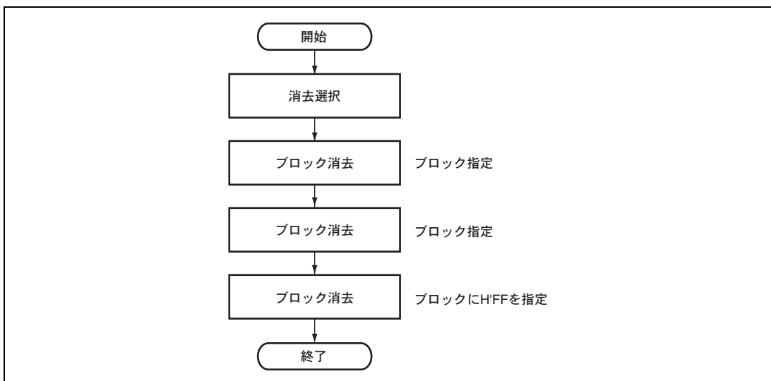
図 25.12 ブートモードでの ROM 消去方法
