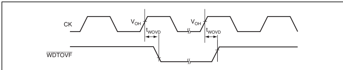
図 32.17 ウォッチドッグタイマタイミング
