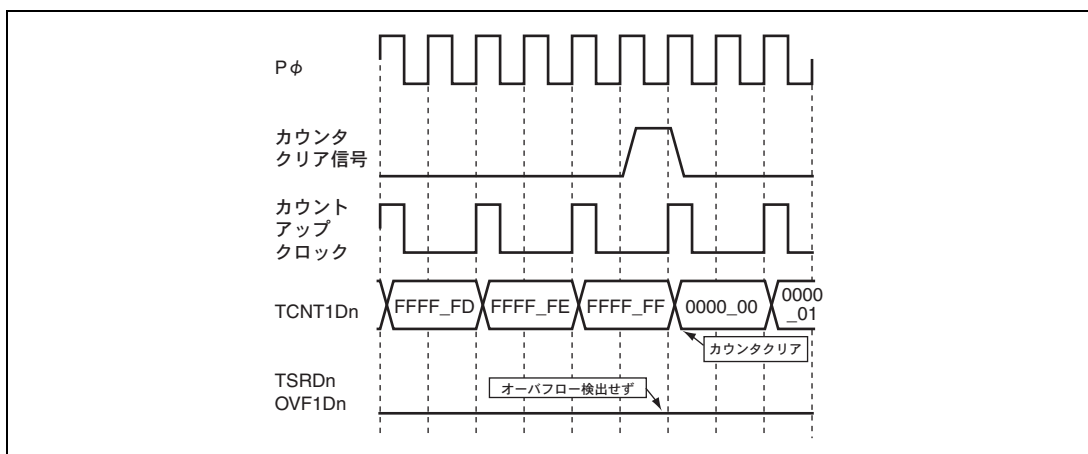
図 13.82 カウンタクリアとオーバーフローの競合
