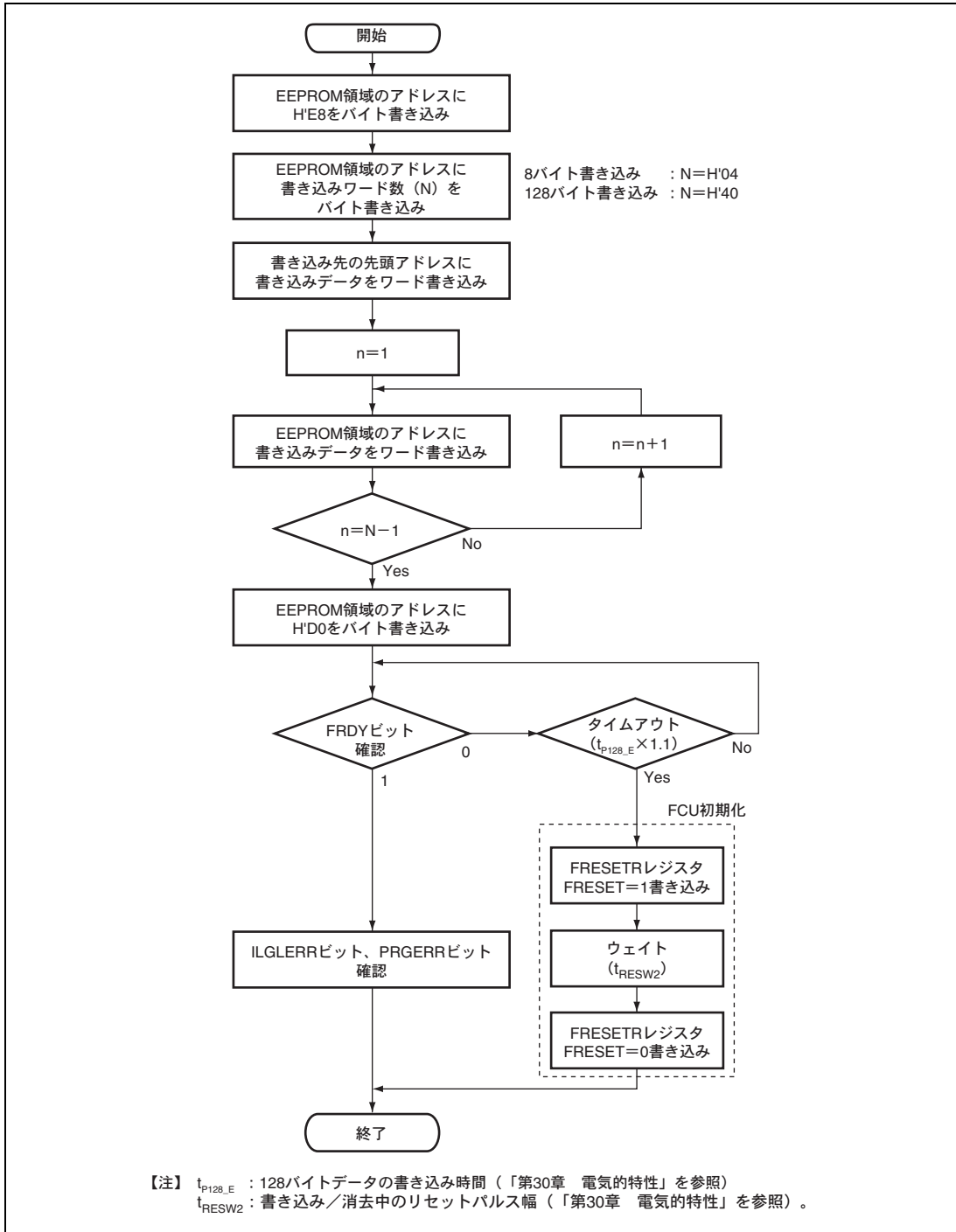
図 26.6 EEPROM の書き込み
