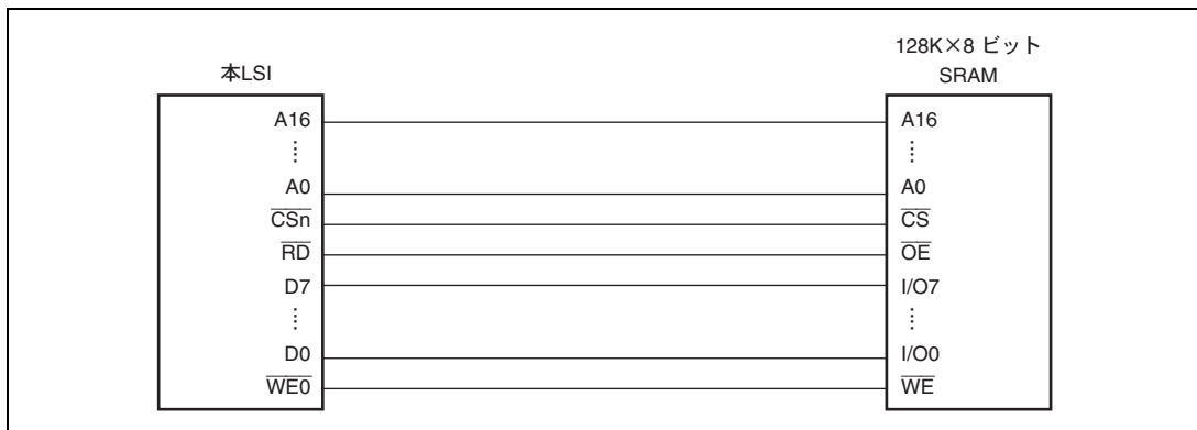
図 10.8 8 ビットデータ幅 SRAM 接続例
