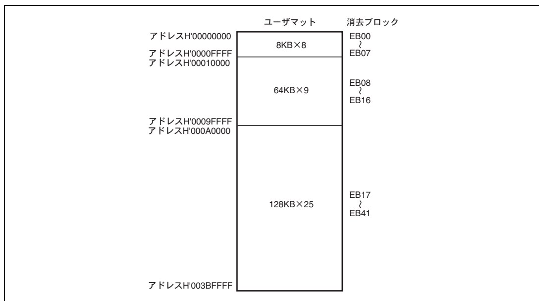
図 25.3 ユーザマットのブロック分割
