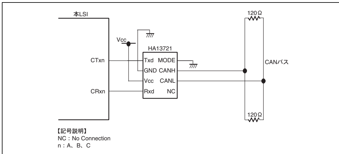
図 18.30 HA13721 を用いた高速 CAN インタフェース
