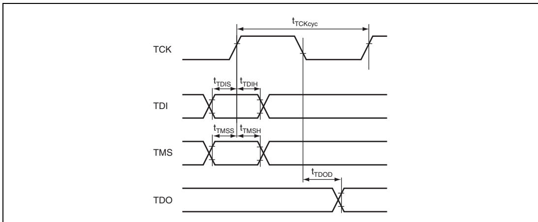
図 32.32 JTAG インタフェース入出力タイミング
