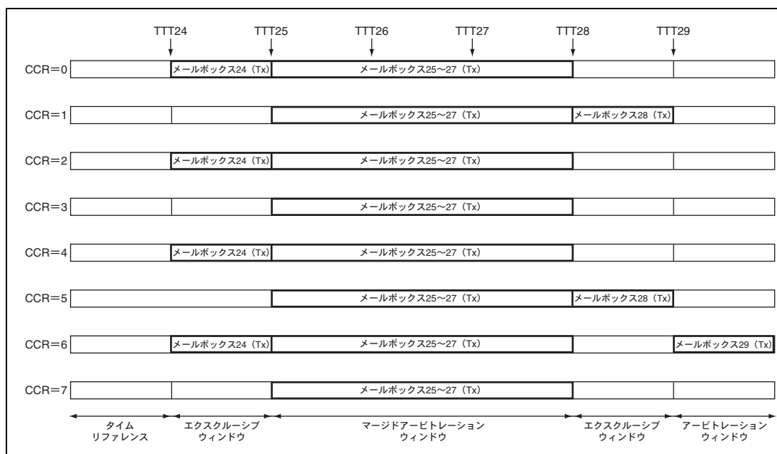
図 18.24 タイムスレープとしてのタイムトリガシステム例
