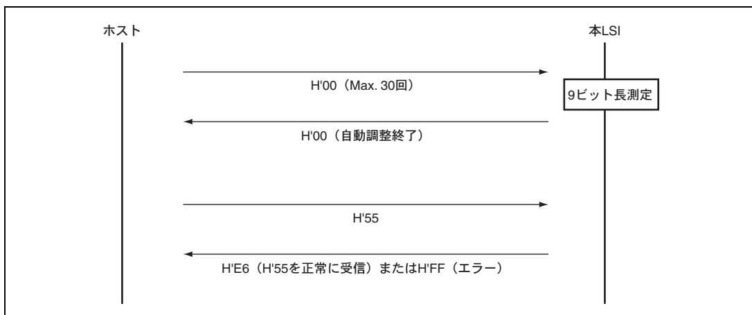
図 25.8 ホストと本 LSI 間の通信シーケンス
