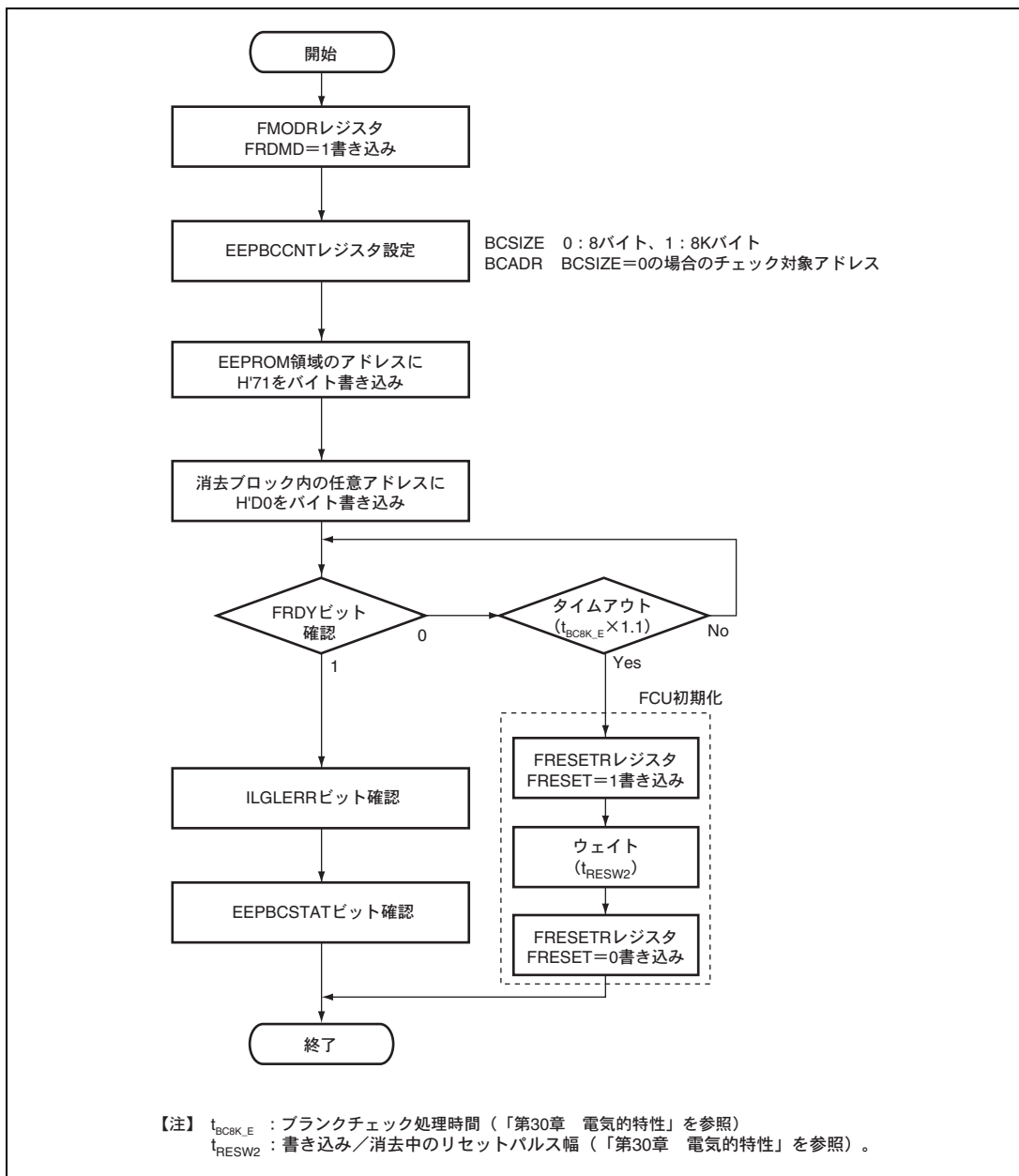
図 26.7 EEPROM のブランクチェック
