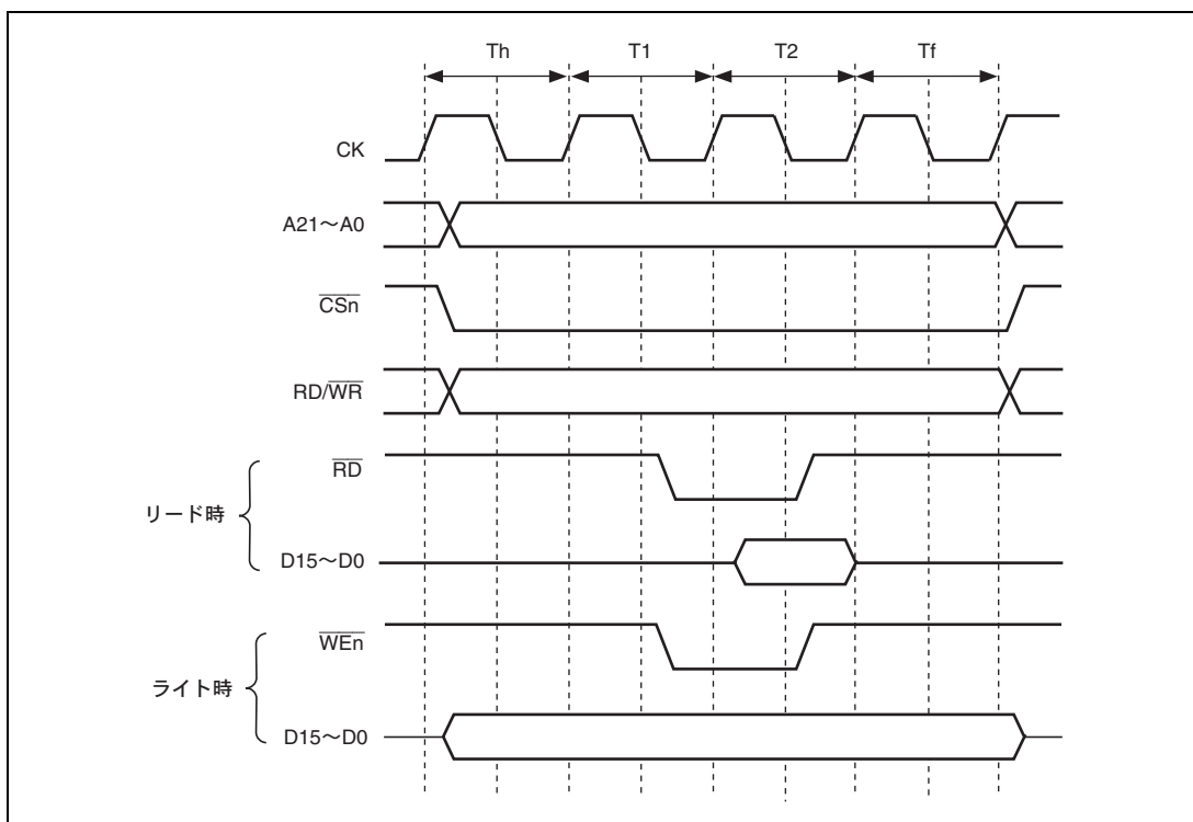
図 10.11 \overline{CSn} アサート期間拡張
