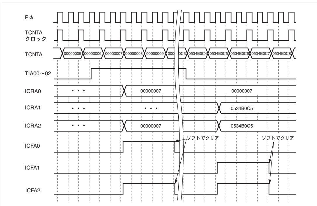
図 13.10 タイマ A のインプットキャプチャ動作
