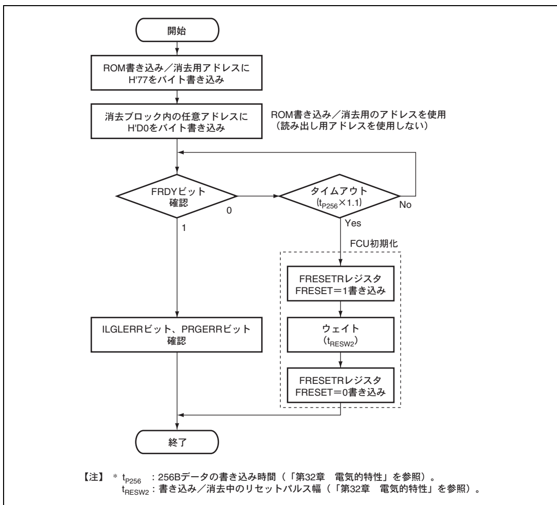
図 25.26 ロックビットのプログラム方法
