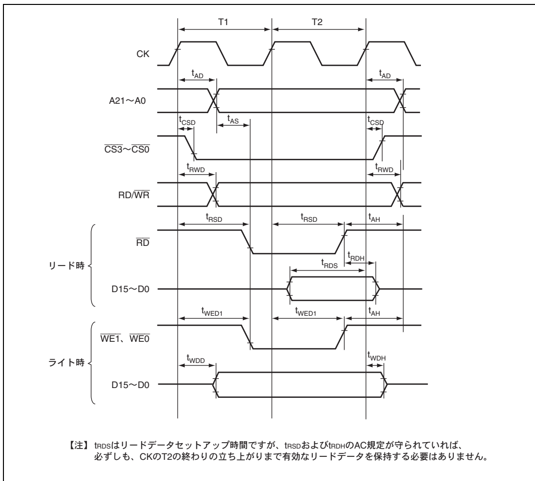
図 32.8 バスサイクル（ノーウェイト）
