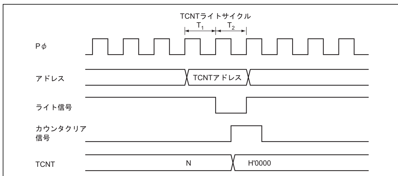
図 9.46 TCNT のライトとクリアの競合
