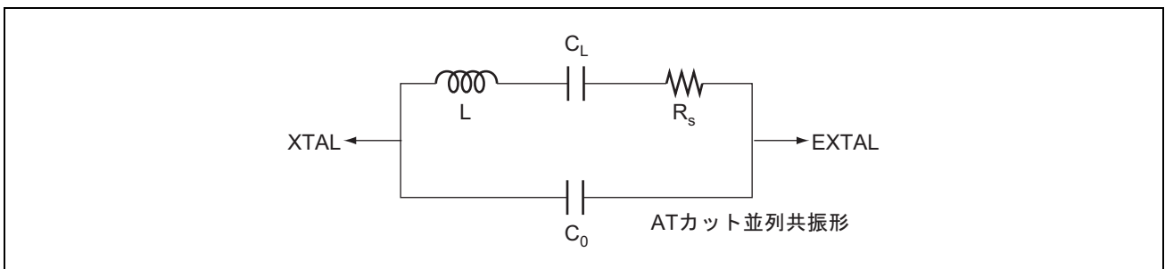
図 17.3 水晶発振子の等価回路
