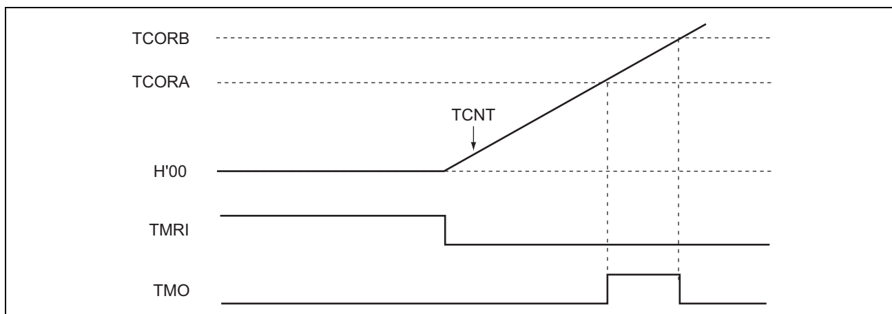
図 11.4 リセット入力例
