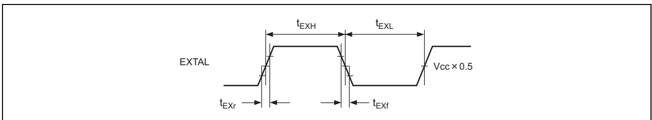
図 20.5 外部入力クロックタイミング
