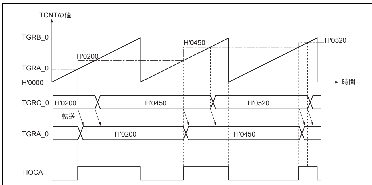
図 9.15 バッファ動作例 (1)
