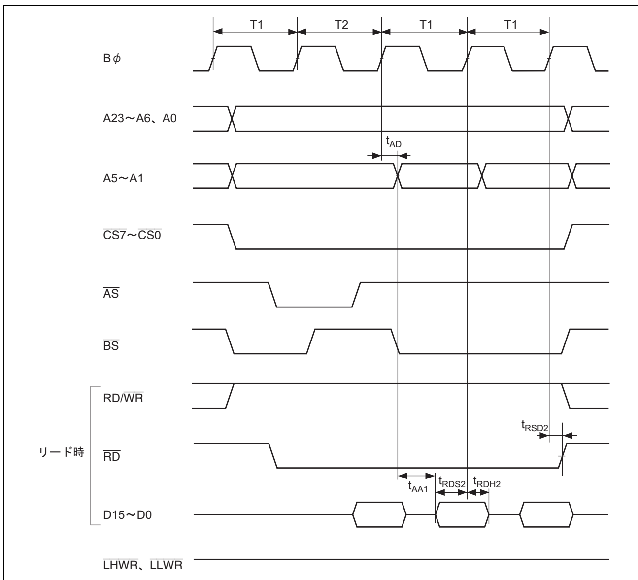
図 20.15 パースト ROM アクセスタイミング／1 ステートパーストアクセス
