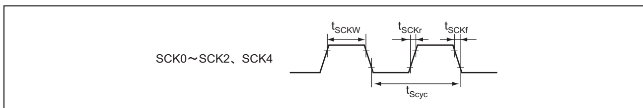
図 20.29 SCK クロック入力タイミング
