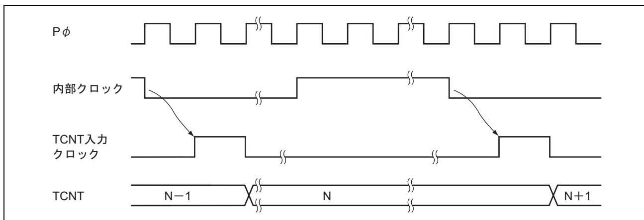
図 11.5 内部クロック立ち下がりエッジ動作時のカウントタイミング
