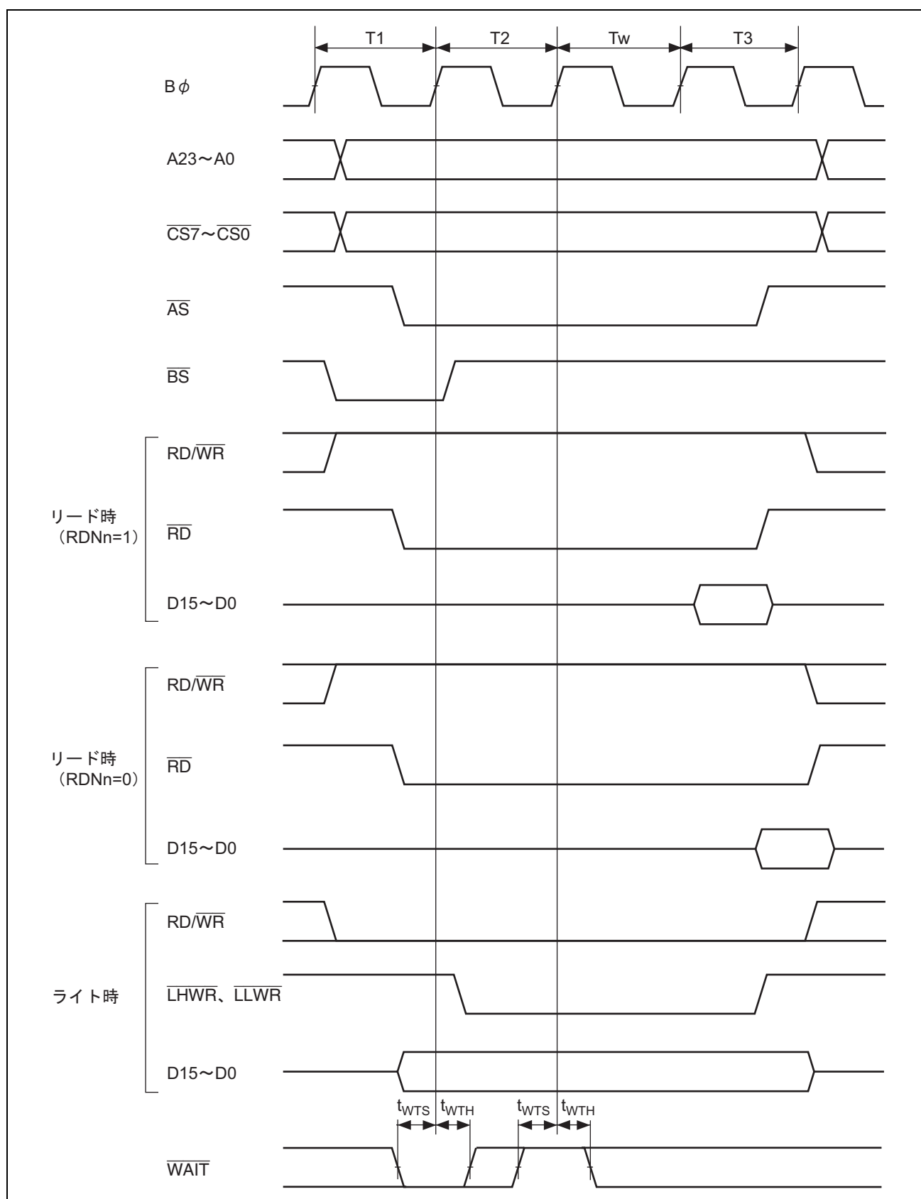
図 20.10 基本バスタイミング/3 ステートアクセス 1 ウェイト
