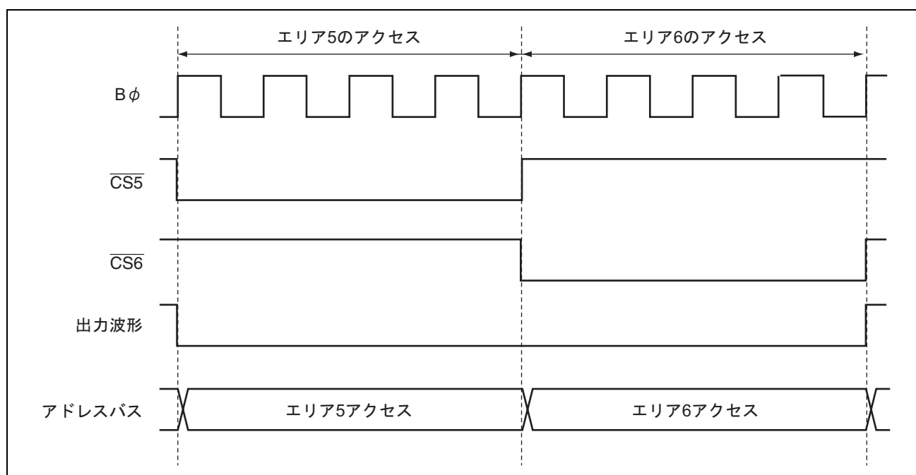
図 6.9 \overline{\text{CS}} を同一端子に出力したときのタイミング
