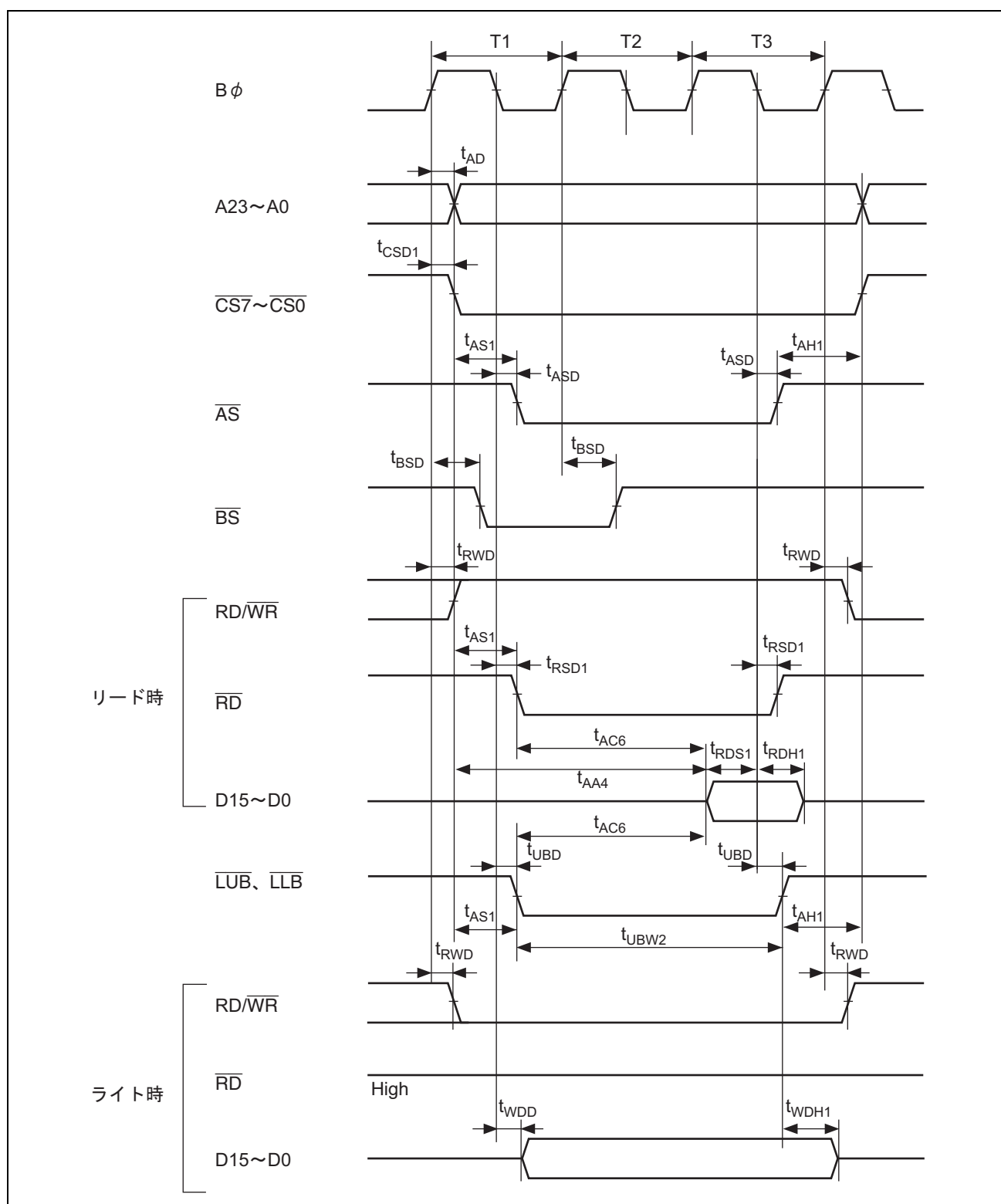
図 20.14 バイト制御 SRAM 3 ステートリード/ライトアクセス
