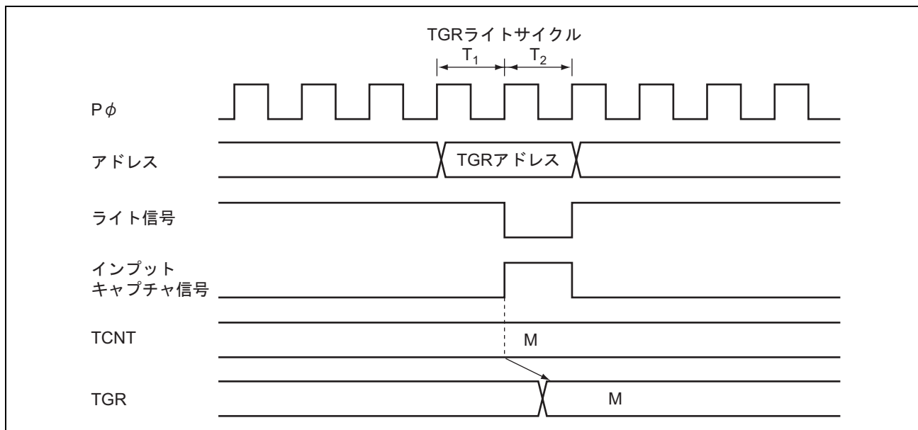
図 9.51 TGR のライトと入力キャプチャの競合
