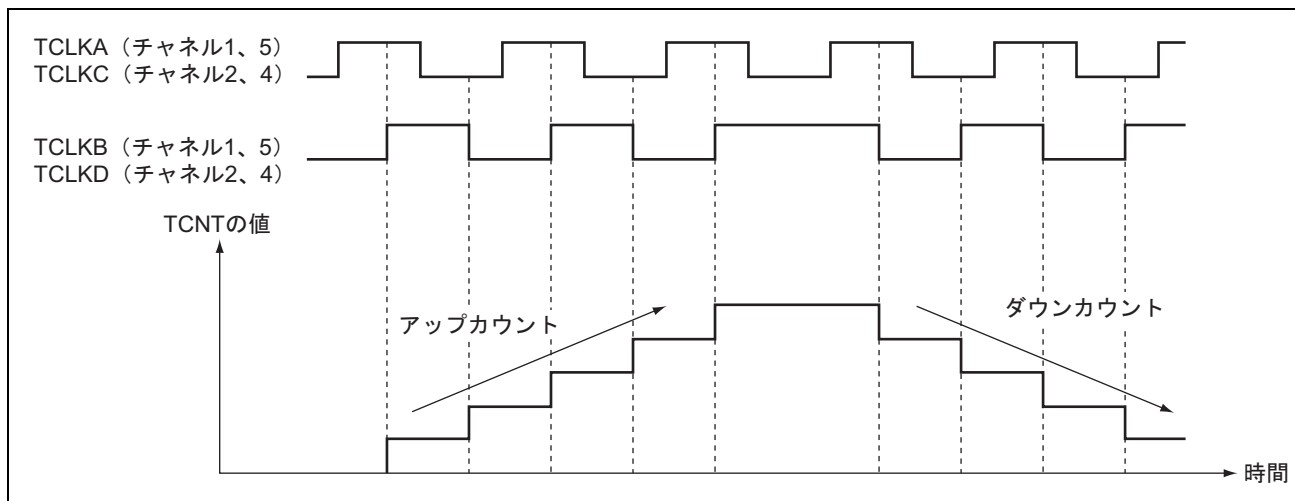
図 9.28 位相計数モード4の動作例
