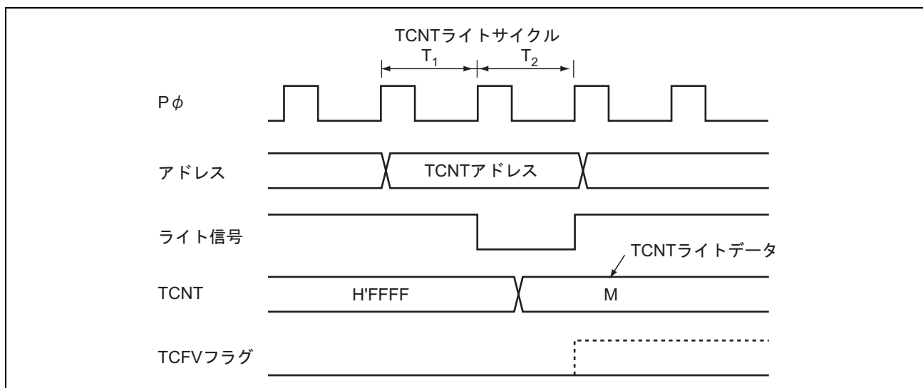
図 9.54 TCNT のライトとオーバフローの競合
