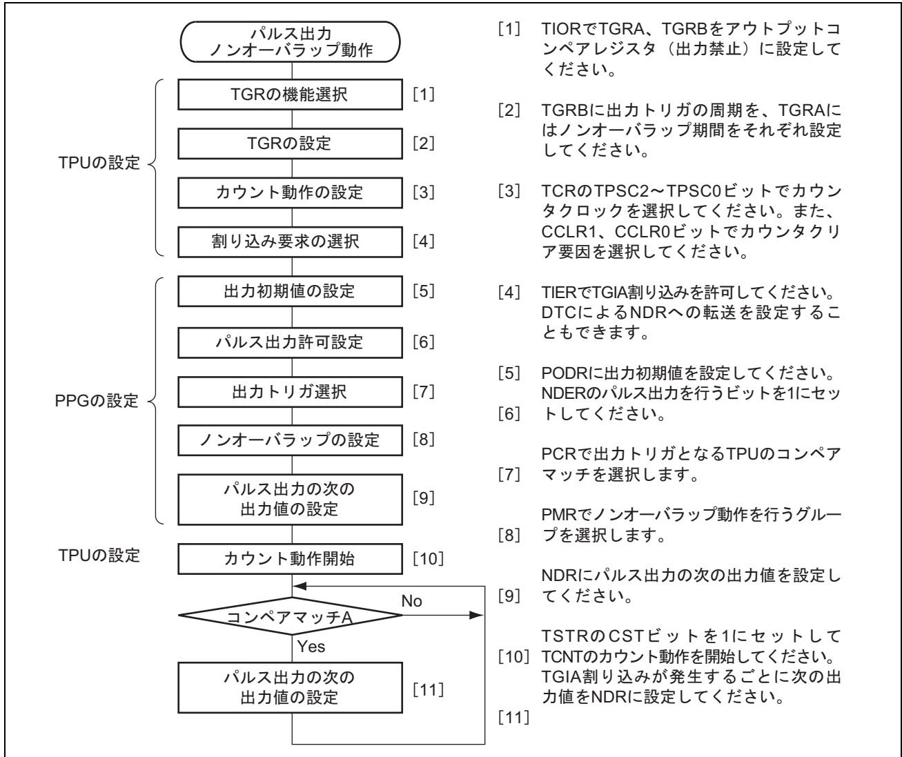
図 10.8 パルス出力ノンオーバーラップ動作の設定手順例
