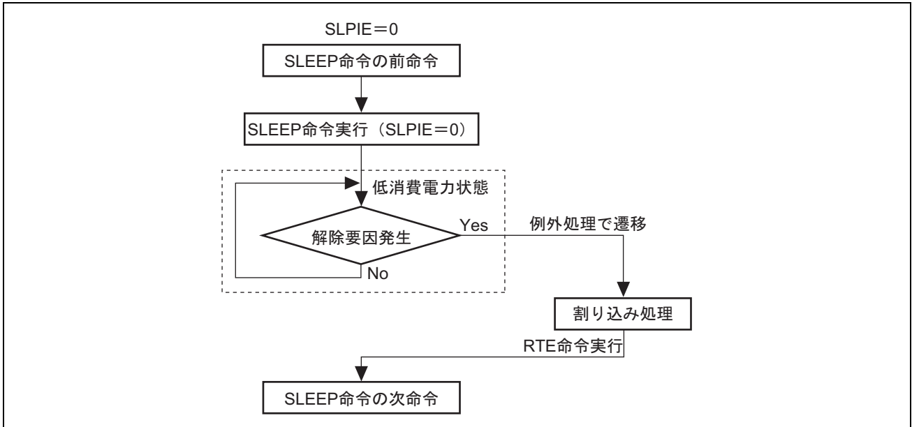
図 18.5 SLEEP 命令実行後に解除要因割り込みが発生した場合
