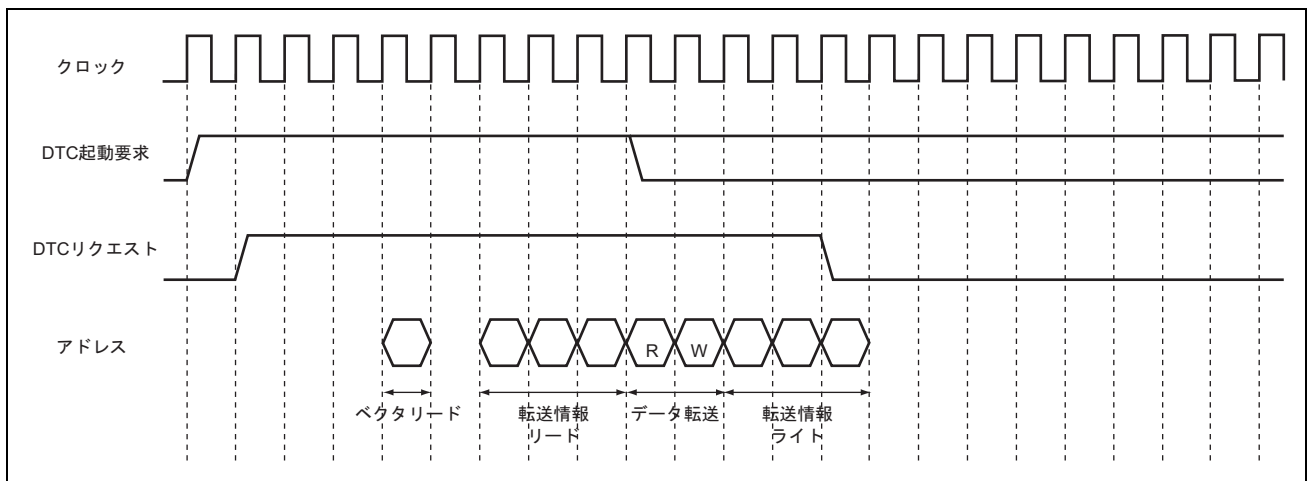
図 7.11 DTC の動作タイミング例 (ショートアドレスモード、ノーマル転送モード、リピート転送モード)
