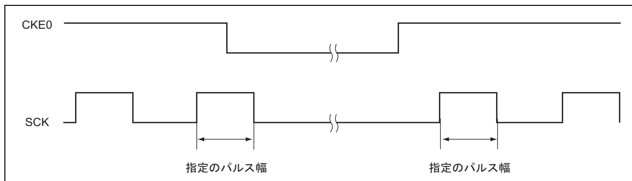
図 13.31 クロック出力固定タイミング
