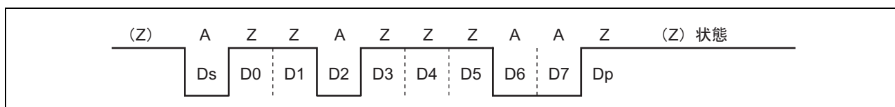
図 13.23 ダイレクトコンベンション (SDIR=SINV=0/E=0)
