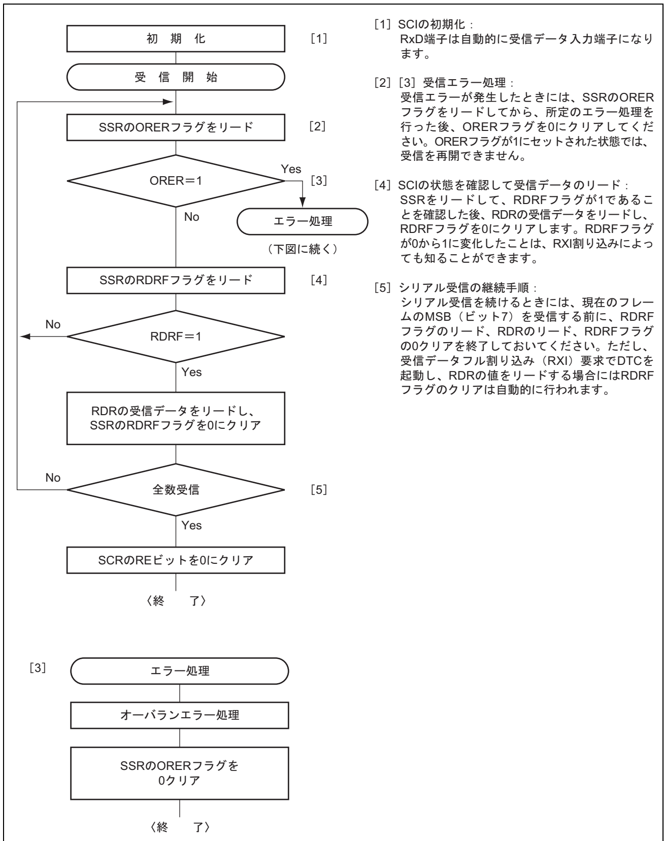
図 13.19 シリアル受信のフローチャートの例
