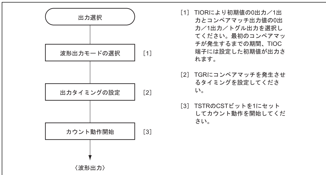
図 9.5 コンペアマッチによる波形出力動作例
