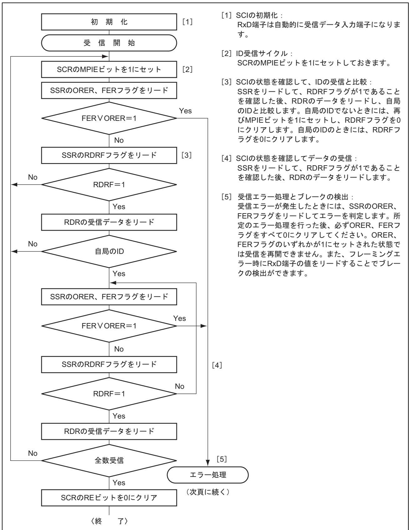
図 13.13 マルチプロセッサシリアル受信のフローチャートの例 (1)
