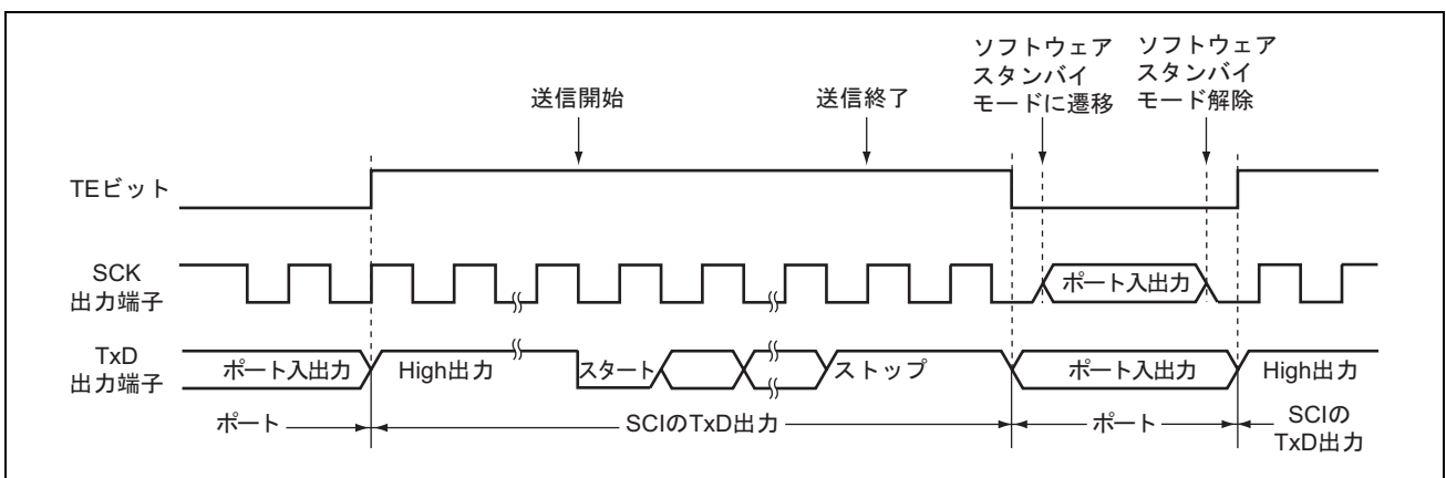
図 13.35 ソフトウェアスタンバイモード遷移時のポートの端子状態 (内部クロック、調歩同期送信)
