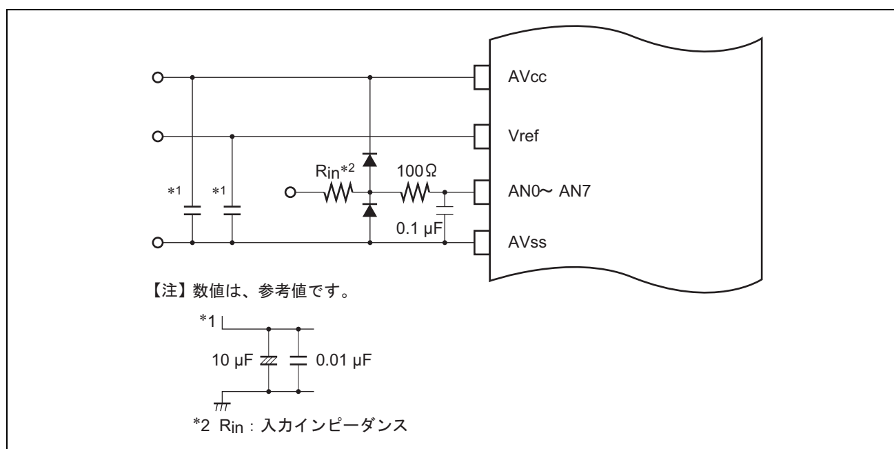
図 14.9 アナログ入力保護回路の例
