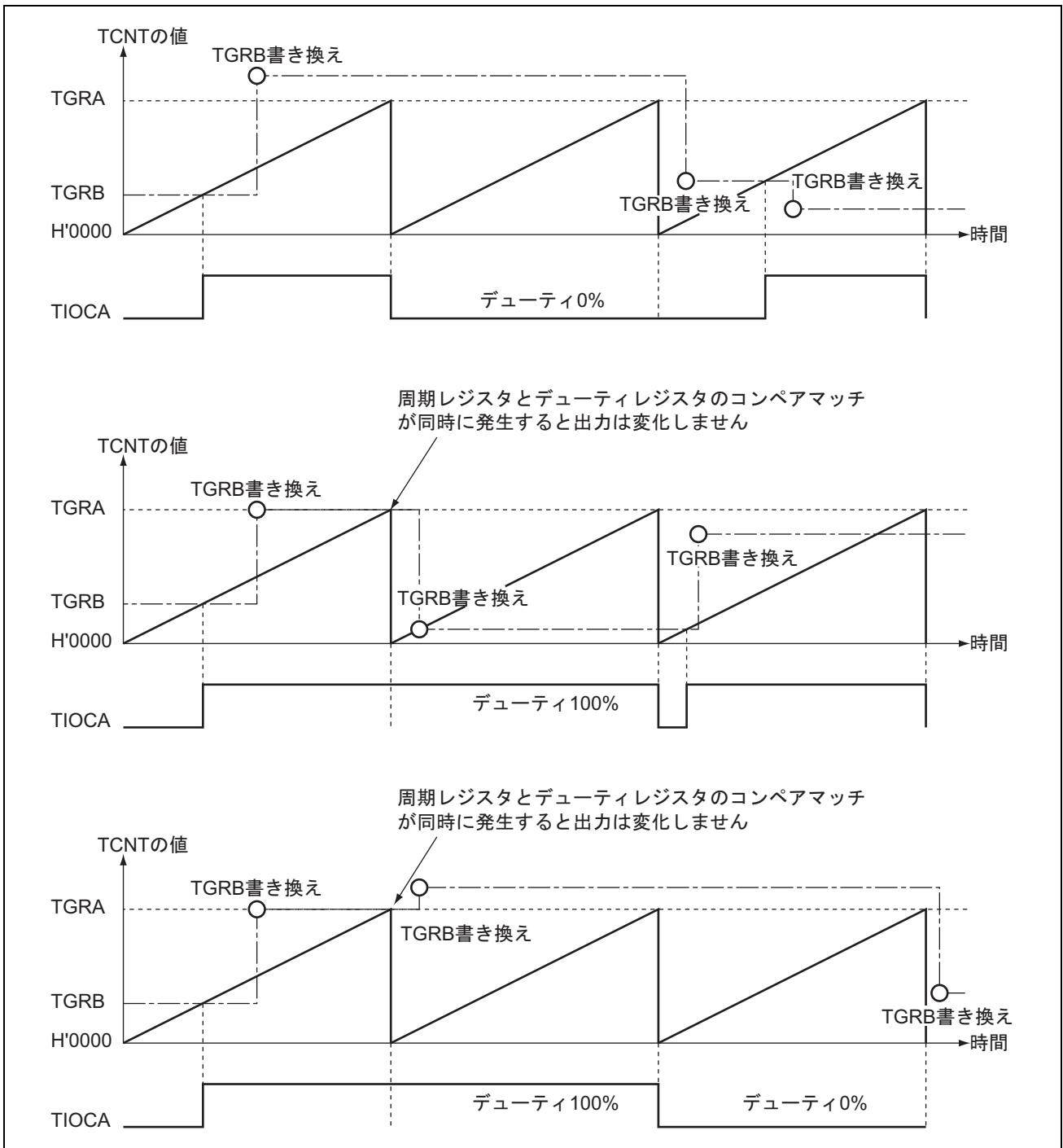
図 9.23 PWM モード動作例 (3)
