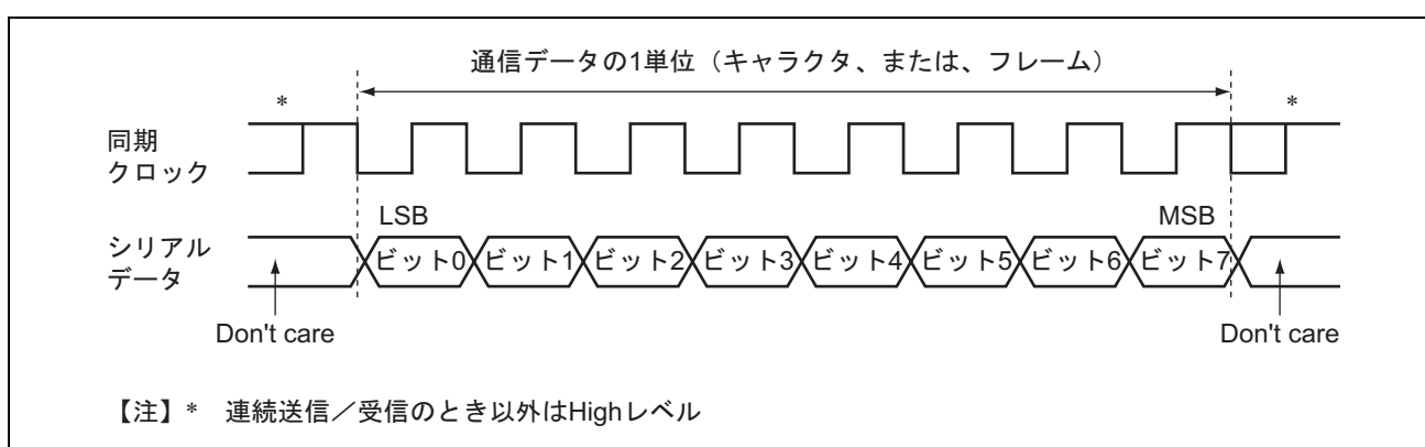
図 13.14 クロック同期式通信のデータフォーマット (LSB ファーストの場合)
