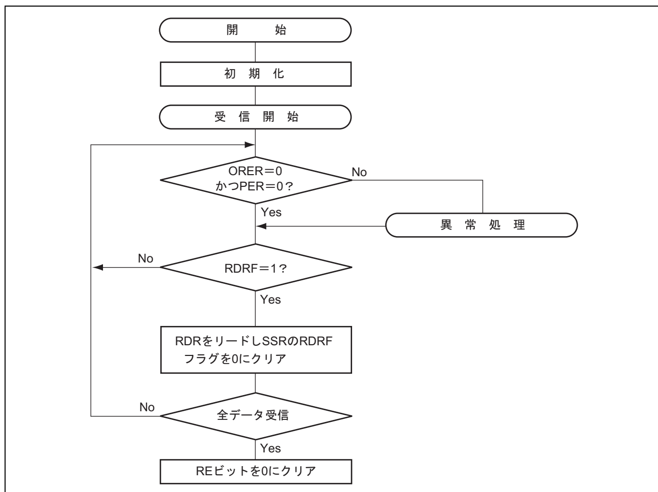
図 13.30 受信フローの例
