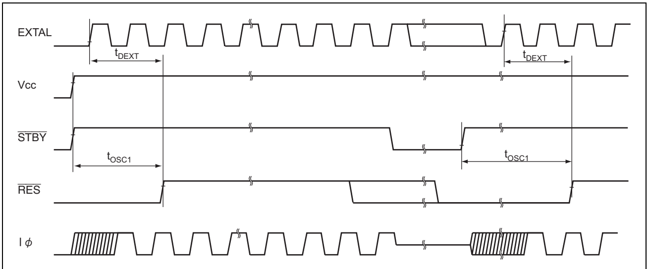
図 20.4 発振安定時間タイミング
