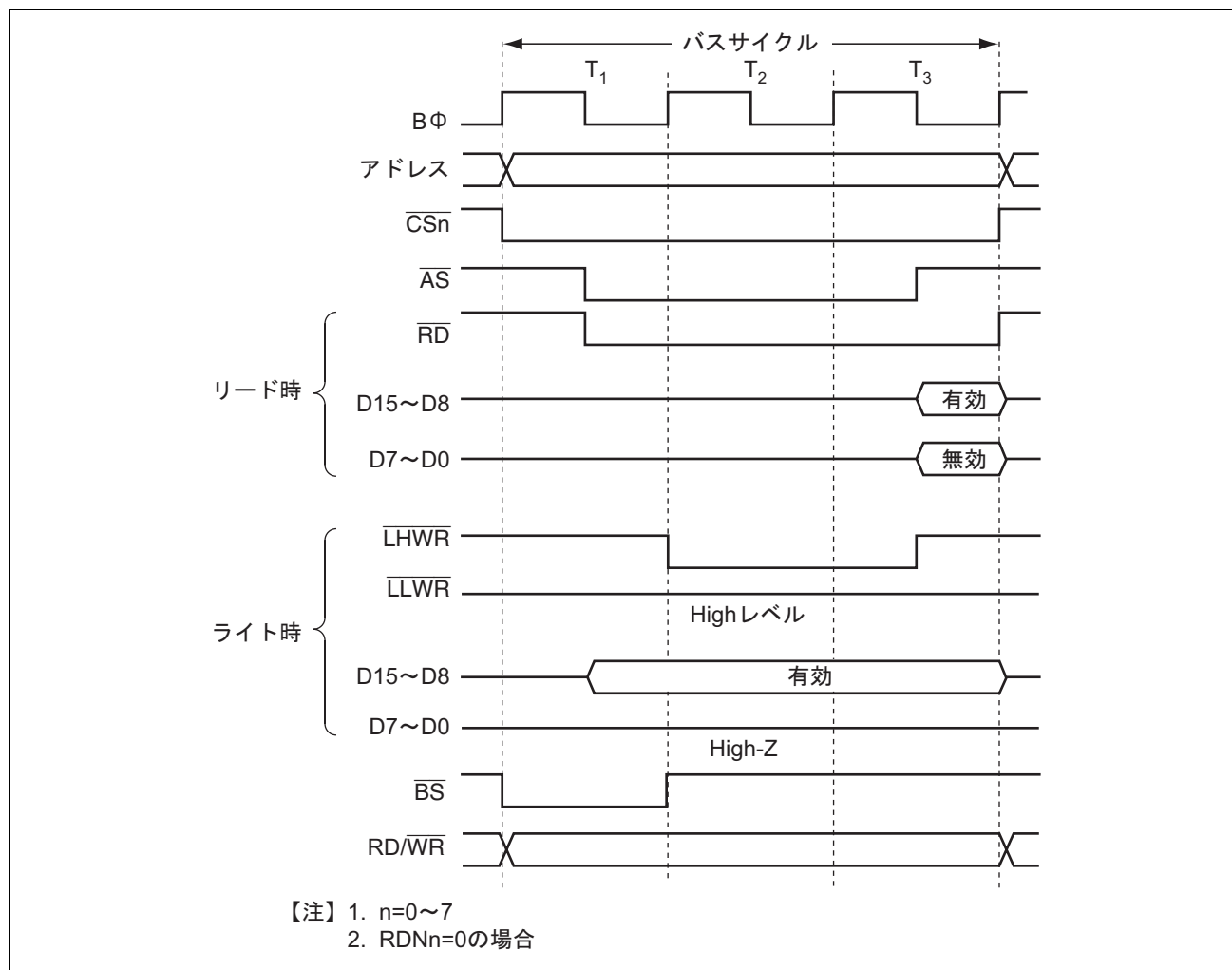
図 6.17 16 ビット 3 ステートアクセス空間のバスタイミング (偶数アドレスバイトアクセス)
