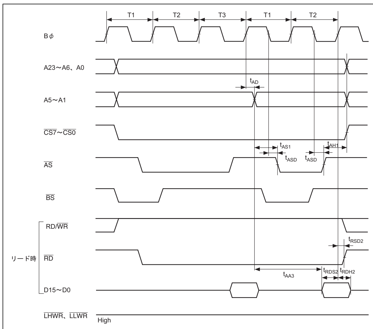
図 20.16 バースト ROM アクセスタイミング/2 ステートバーストアクセス
