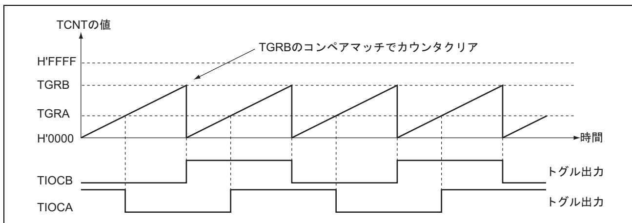
図 9.7 トグル出力の動作例
