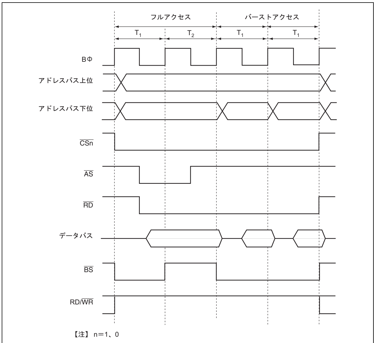
図 6.27 バースト ROM アクセスタイミング例 (ASTn=0、バーストサイクル 1 ステート)
