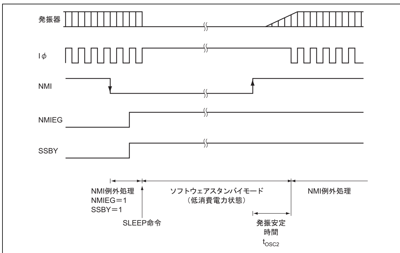
図 18.2 ソフトウェアスタンバイモードの応用例
