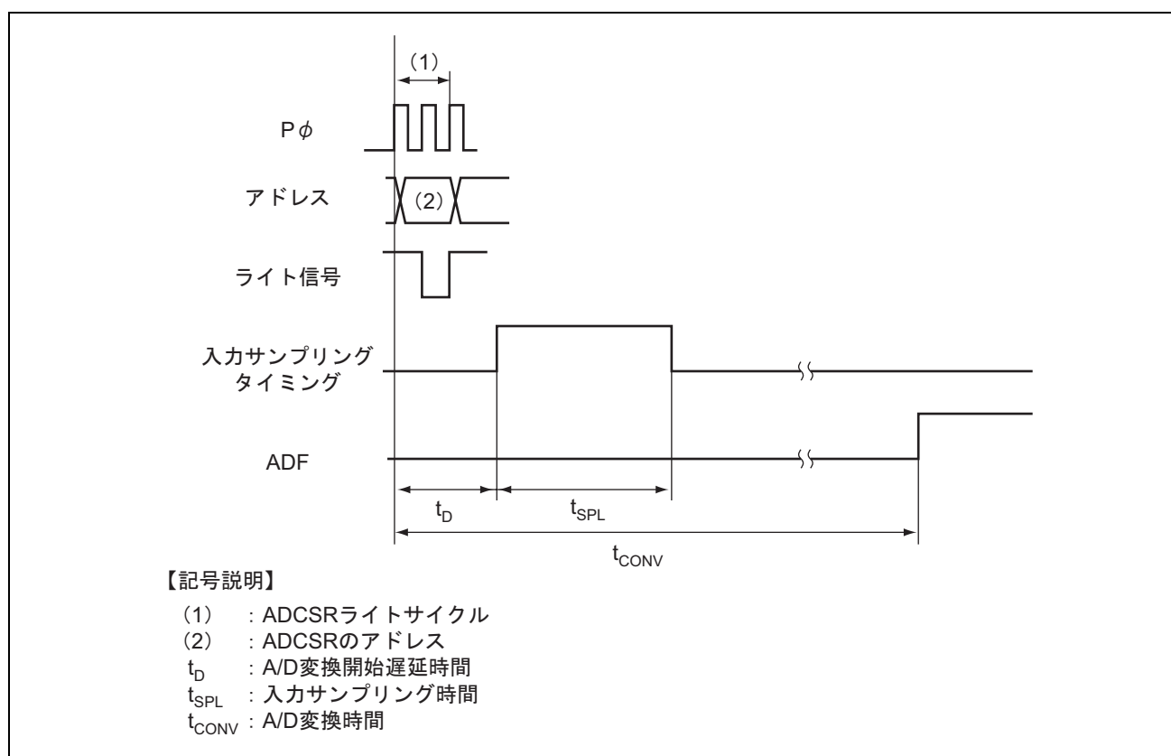
図 14.4 A/D 変換タイミング
