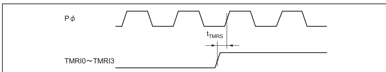
図 20.26 8ビットタイマリセット入力タイミング
