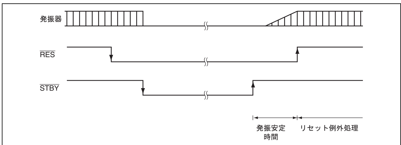
図 18.3 ハードウェアスタンバイモードのタイミング
