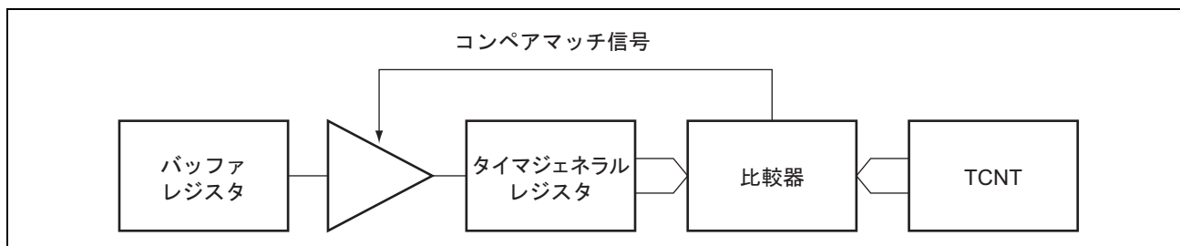
図 9.12 コンペアマッチバッファ動作
