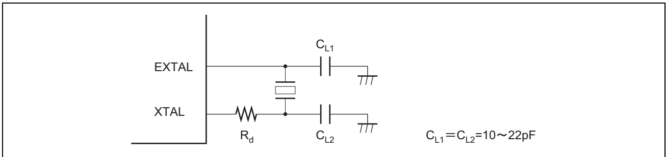
図 17.2 水晶発振子の接続例
