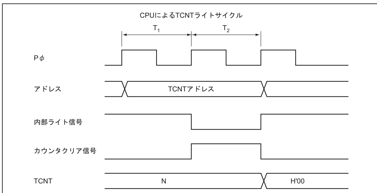
図 11.13 TCNTのライトとクリアの競合
