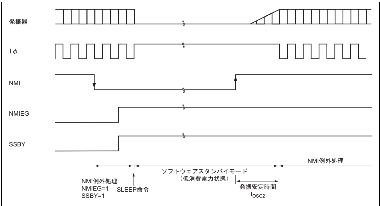
図 20.3 ソフトウェアスタンバイ発振安定時間タイミング
