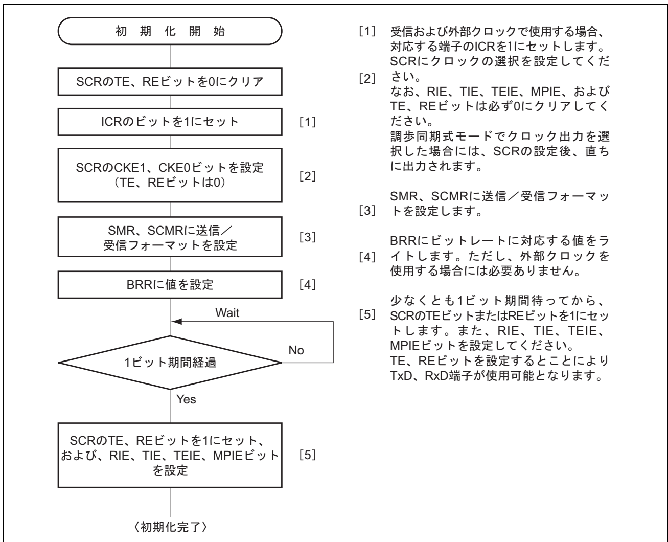
図 13.5 SCI の初期化フローチャートの例
