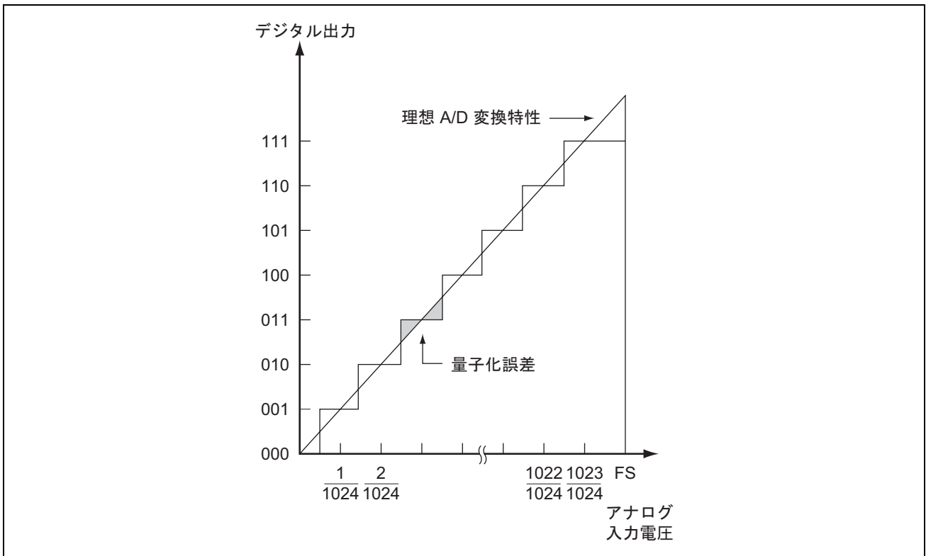
図 14.6 A/D 変換精度の定義
