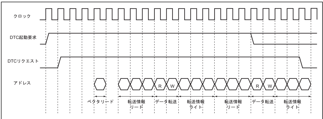
図 7.13 DTC の動作タイミング例 (ショートアドレスモード、チェイン転送)
