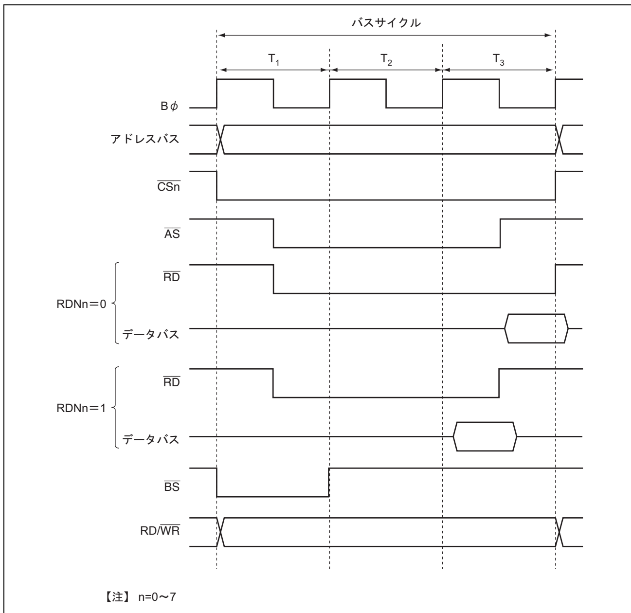
図 6.21 リードストローブタイミング例
