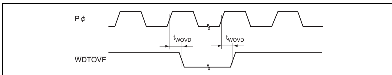
図 20.28 WDT 出力タイミング
