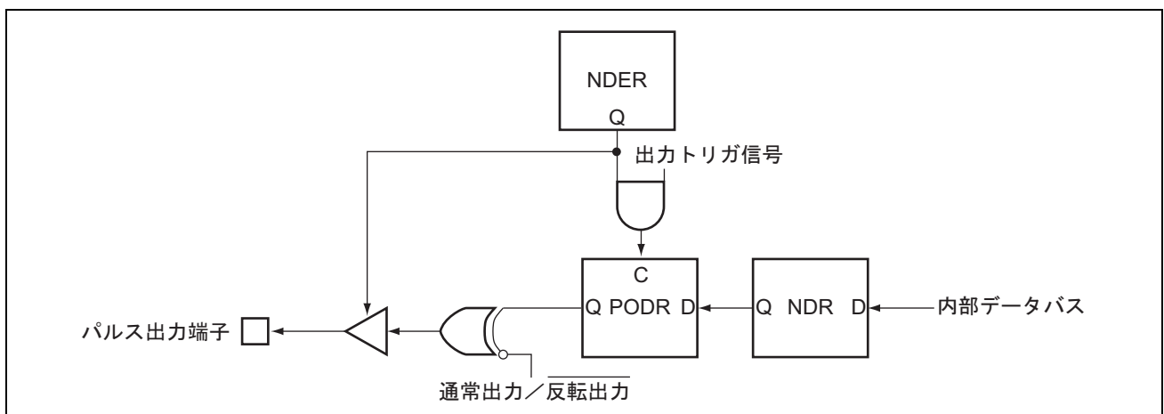
図 10.2 PPG 概要図
