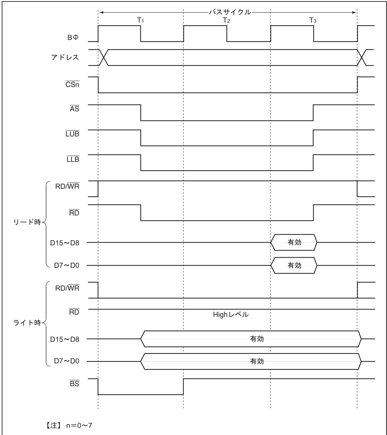
図 6.24 16 ビット 3 ステートアクセス空間のバスタイミング
