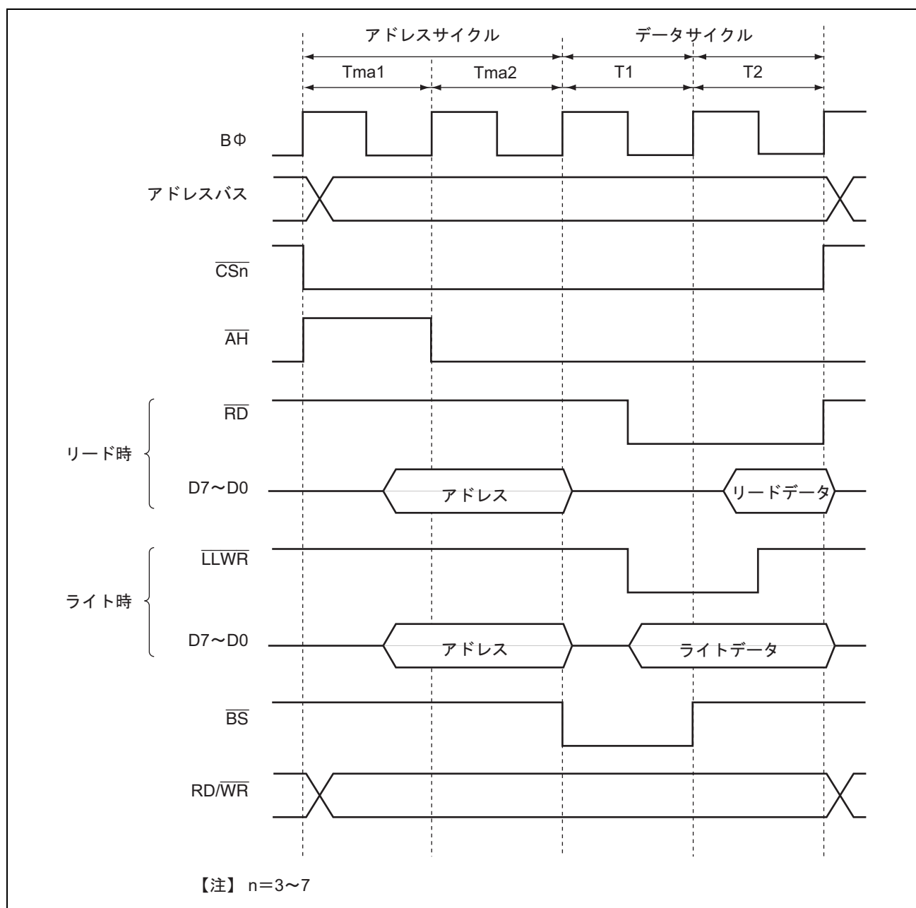
図 6.28 8 ビットアクセス空間へのアクセスタイミング (ABWHn=1、ABWLn=1)
