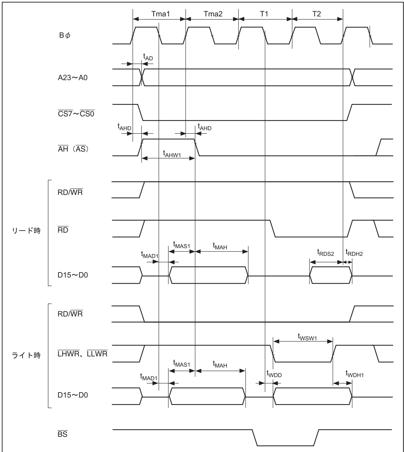
図 20.17 アドレス/データマルチプレクス・アクセスタイミング (ノーウェイト) (-基本・4 ステートアクセス)
