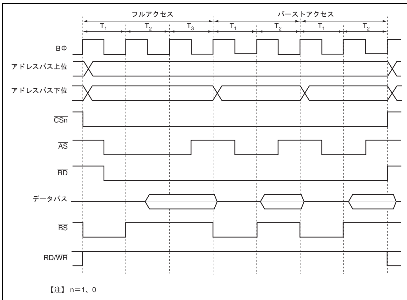
図 6.26 バースト ROM アクセスタイミング例 (ASTn=1、バーストサイクル 2 ステート)
