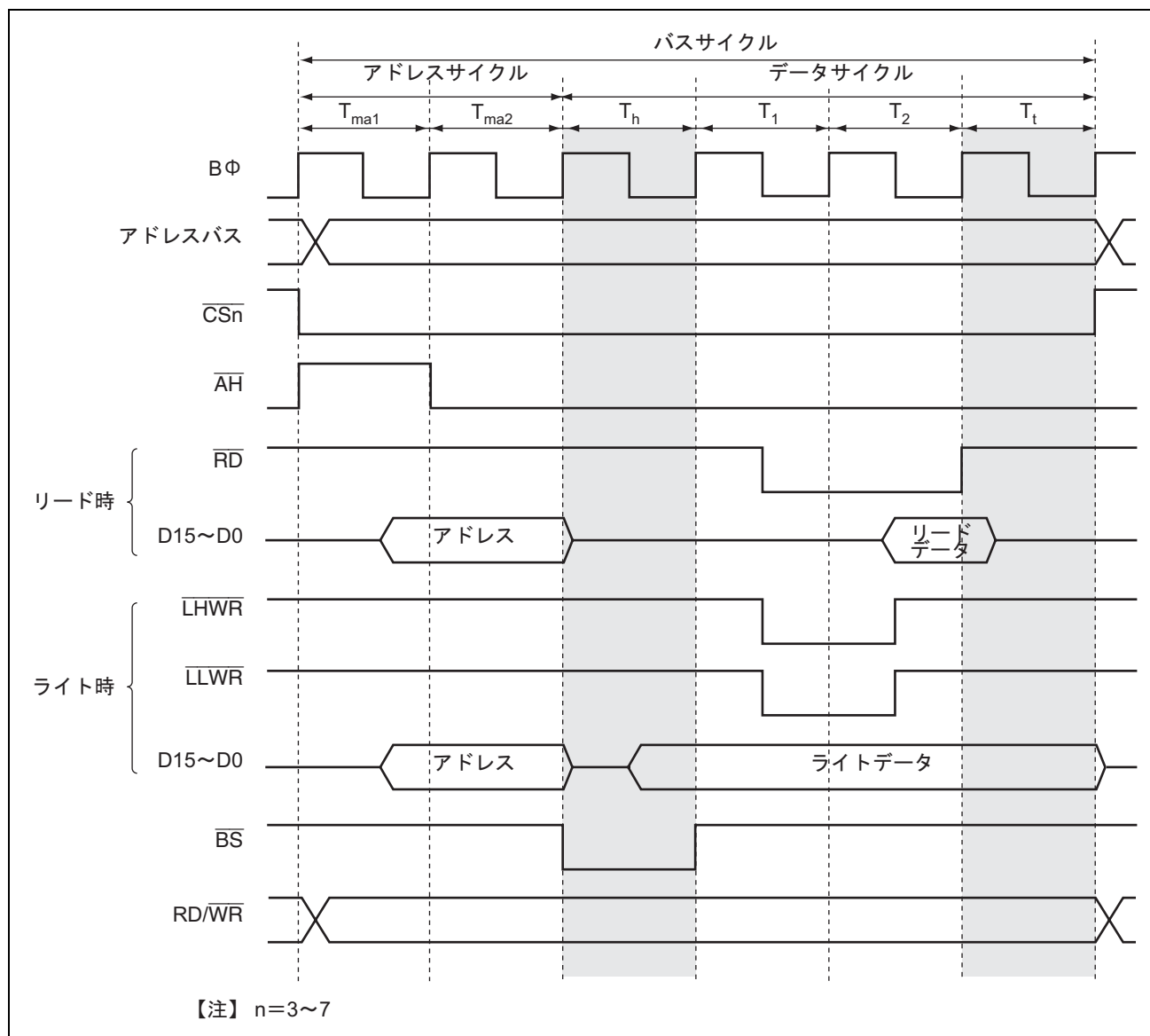
図 6.32 データサイクルのチップセレクトアサート期間拡張タイミング例
