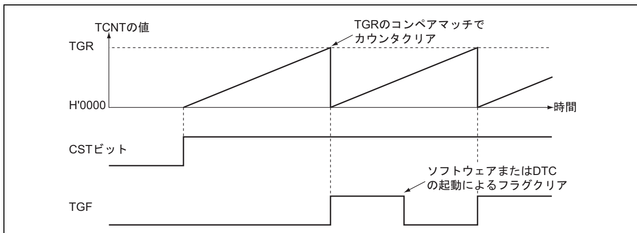
図 9.4 周期カウンタの動作
