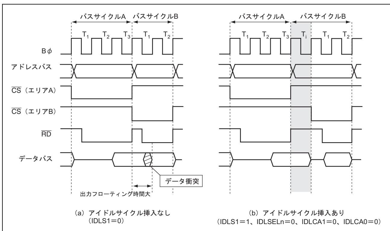
図 6.34 アイドルサイクル動作例 (異なるエリア間での連続リード)
