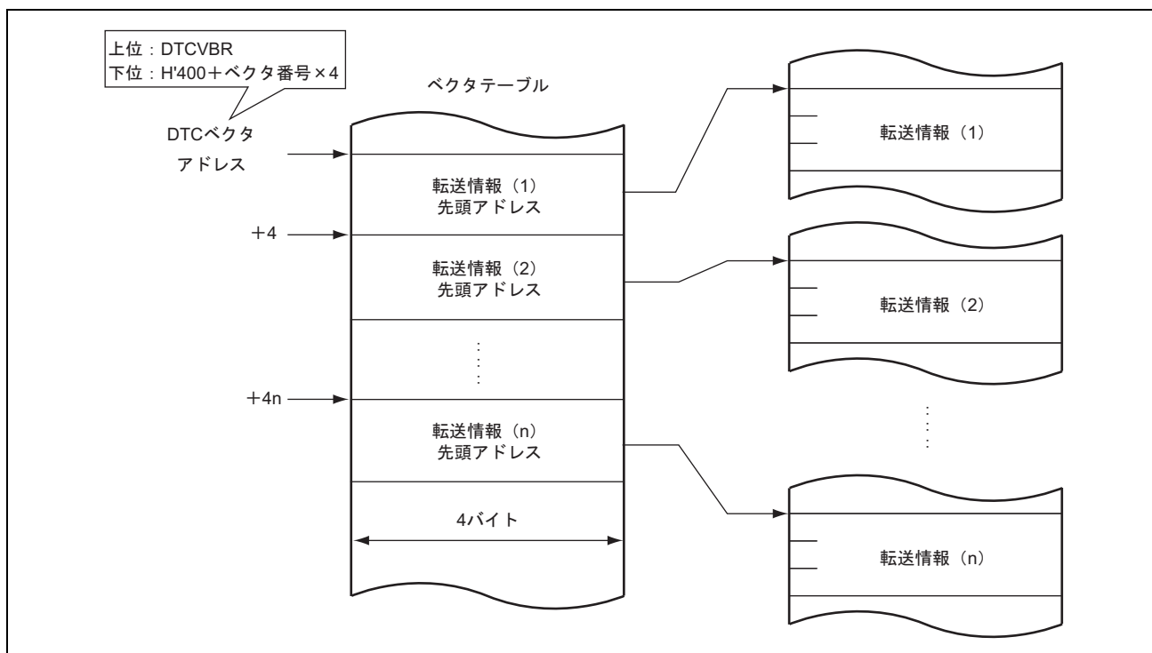
図 7.3 DTC ベクタテーブルと転送情報の対応
