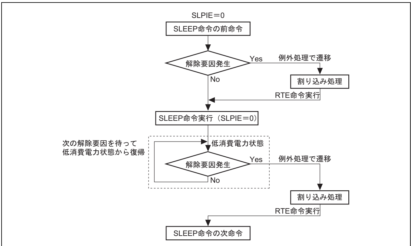
図 18.6 SLEEP 命令実行直前に解除要因割り込みが発生した場合 (スリープ命令例外処理が発生しない場合)
