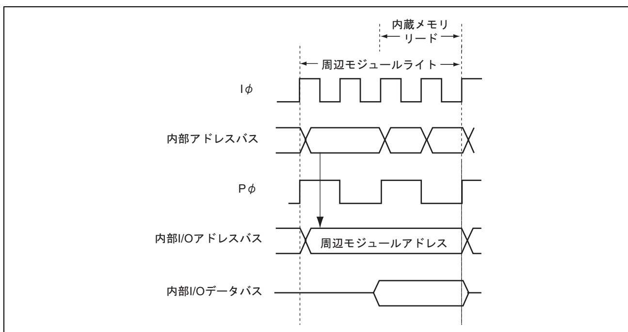
図 6.41 周辺モジュールライトデータバッファ機能使用時のタイミング例
