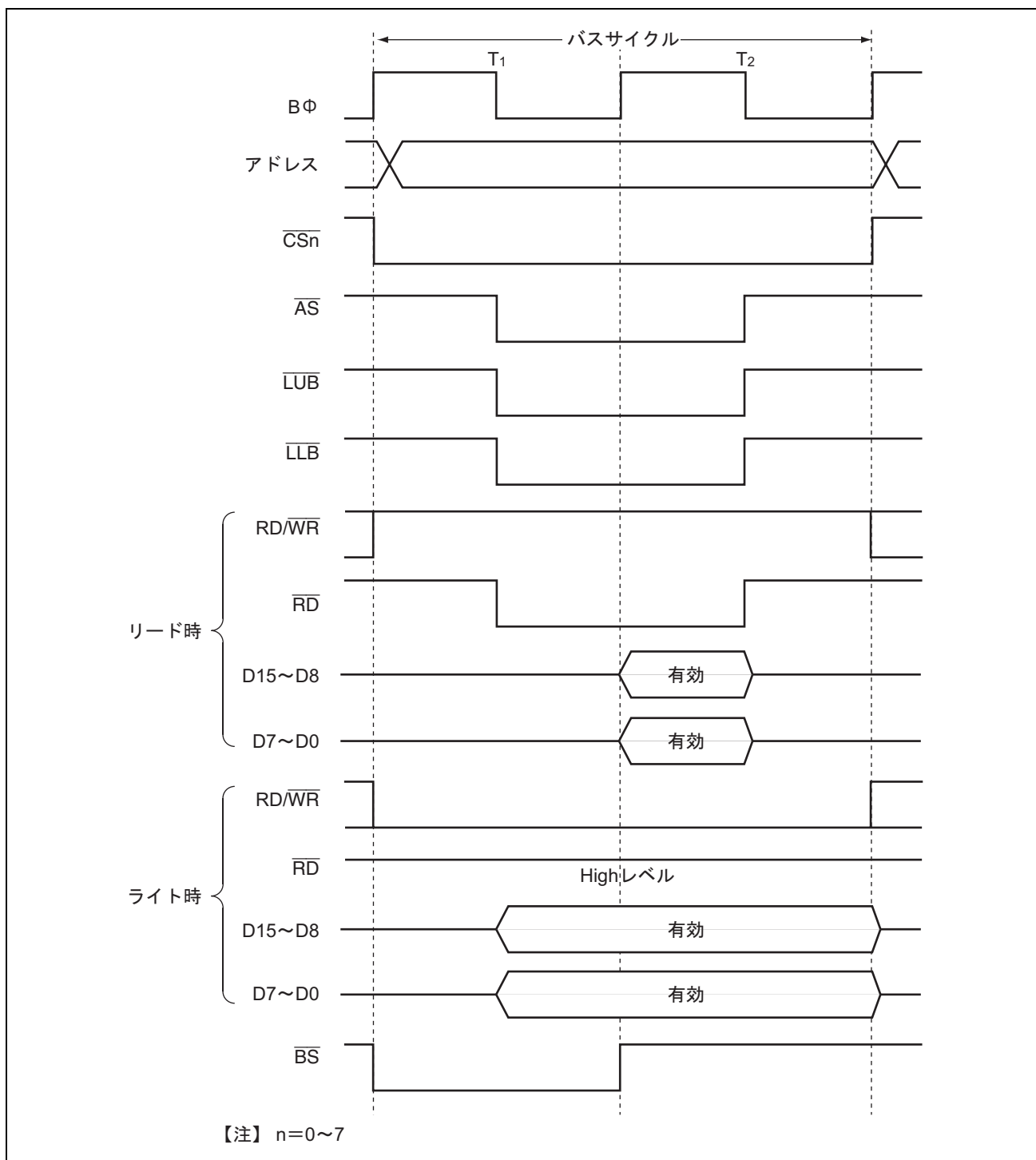
図 6.23 16 ビット 2 ステートアクセス空間のバスタイミング
