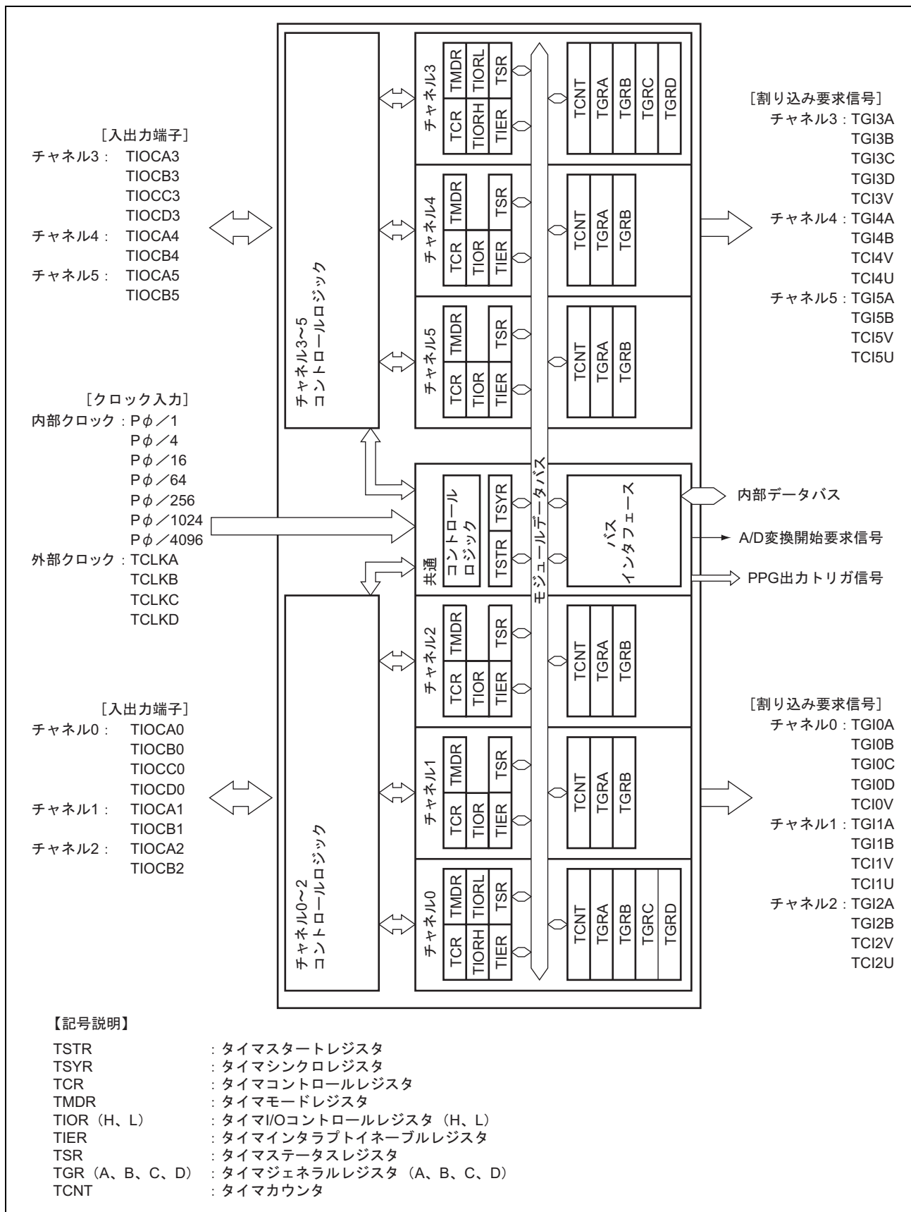
図 9.1 TPU のブロック図
