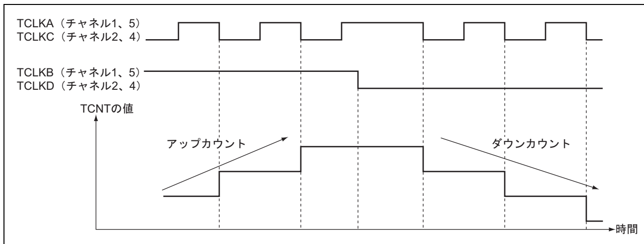
図 9.26 位相計数モード2の動作例
