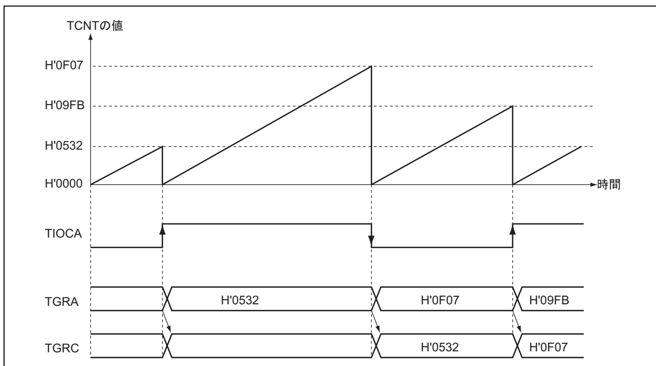
図 9.16 バッファ動作例 (2)
