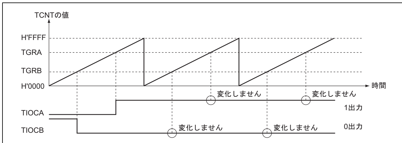
図 9.6 0出力/1出力の動作例
