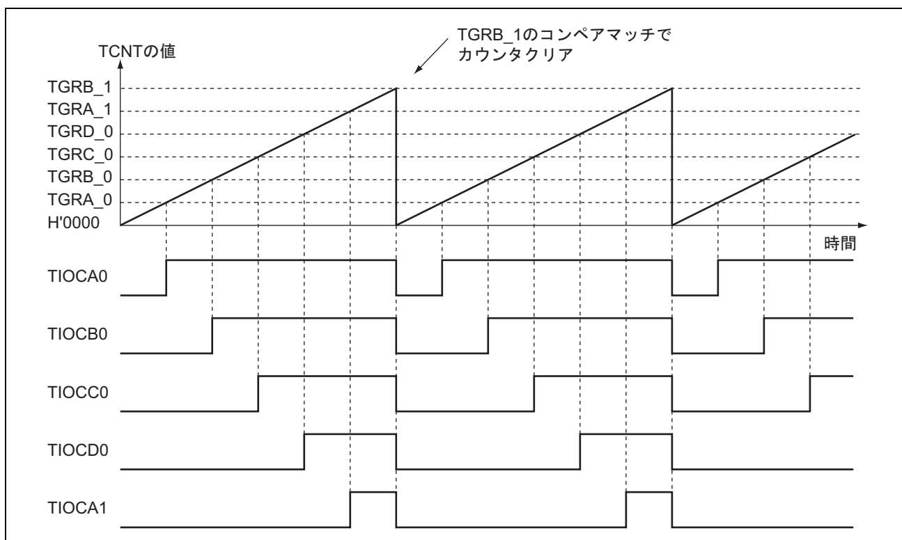
図 9.22 PWM モードの動作例 (2)
