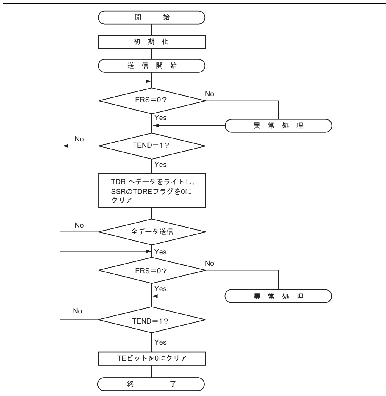
図 13.28 送信処理フローの例
