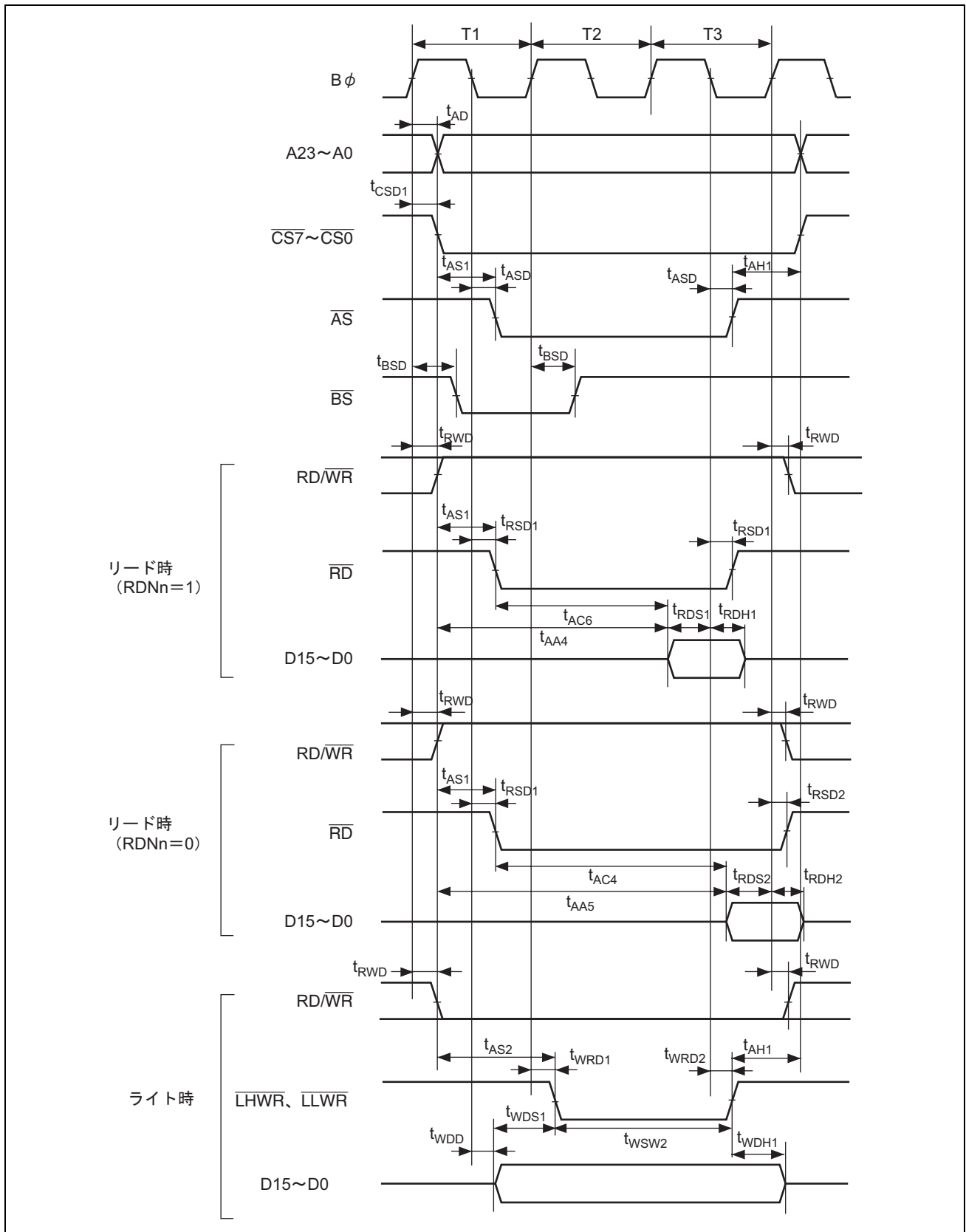
図 20.9 基本バスタイミング/3 ステートアクセス
