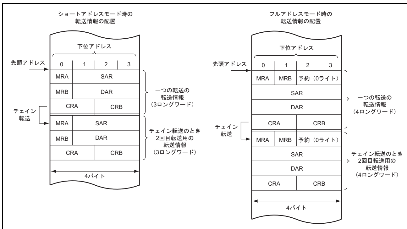
図 7.2 データ領域上での転送情報の配置
