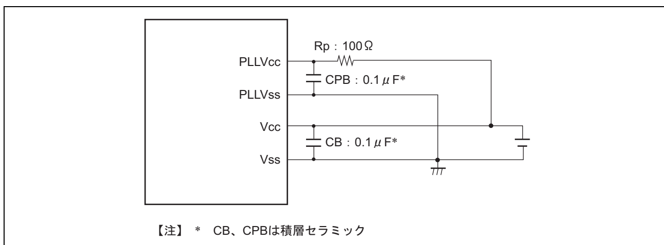
図 17.7 PLL 回路の外付け推奨回路
