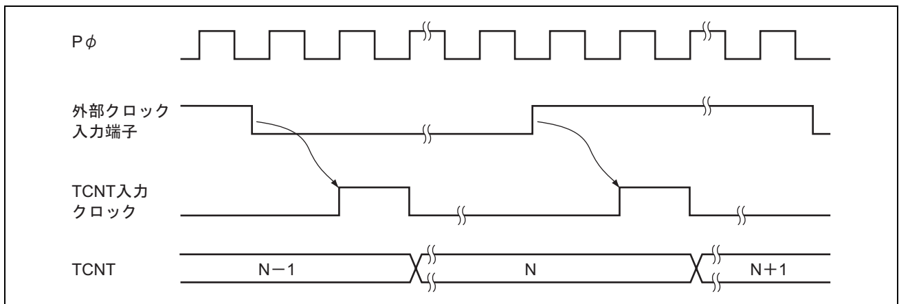
図 11.6 外部クロック立ち上がりエッジ、立ち下がり両エッジ動作時のカウントタイミング
