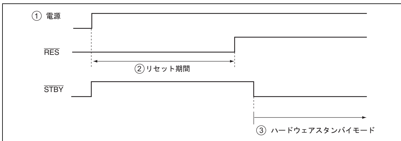
図 18.4 電源投入時のタイミング
