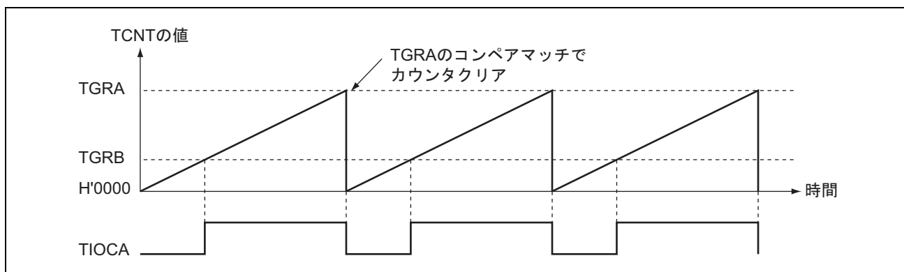
図 9.21 PWM モードの動作例 (1)
