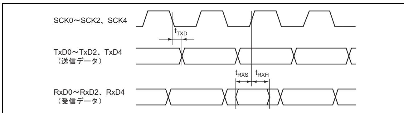
図 20.30 SCI 入出力タイミング/クロック同期式モード
