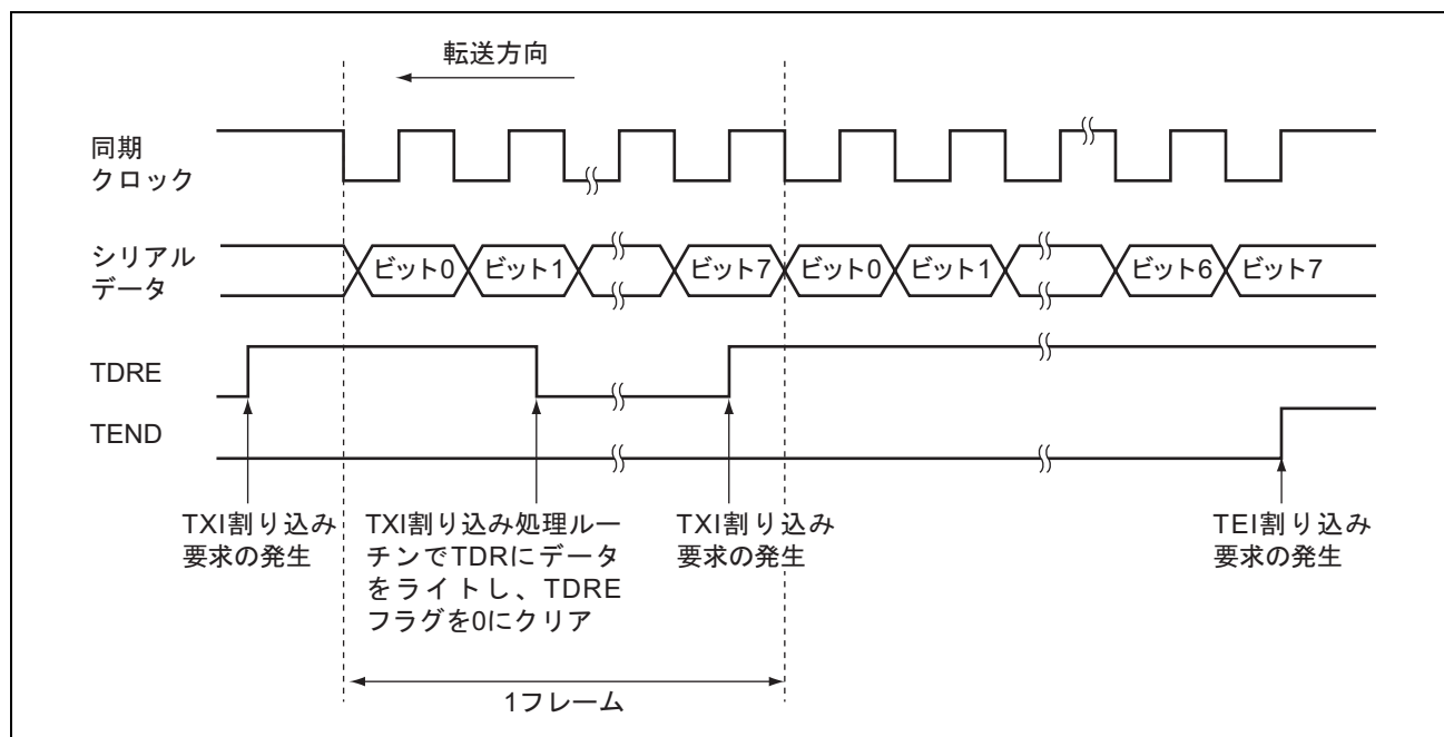
図 13.16 クロック同期式モードの送信時の動作例
