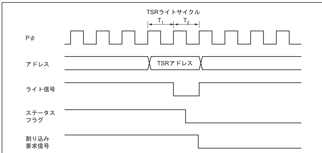
図 9.42 CPUによるステータスフラグのクリアタイミング
