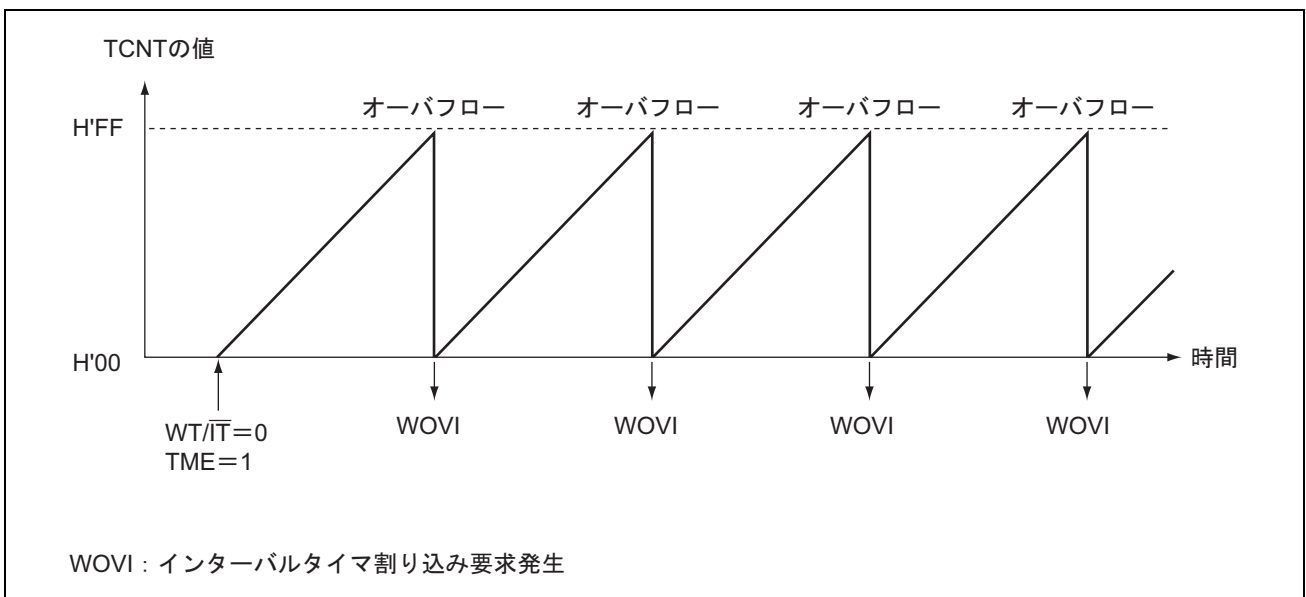
図 12.3 インターバルタイマモード時の動作
