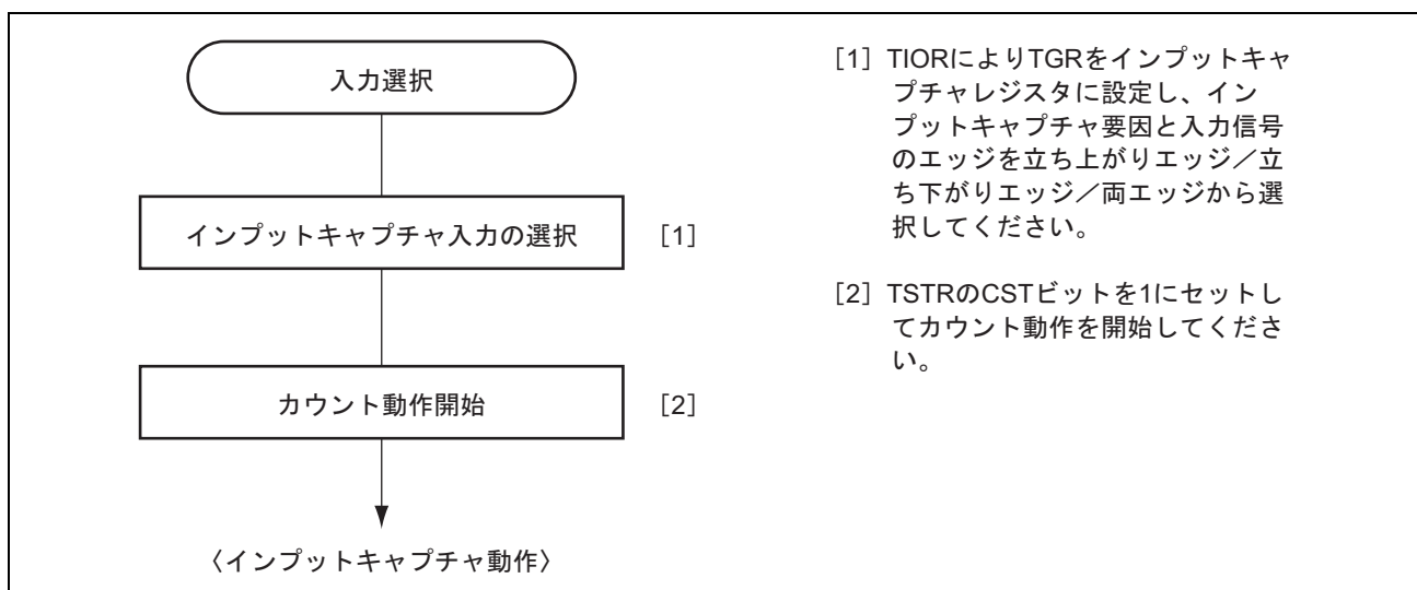
図 9.8 インพุットキャプチャ動作の設定例
