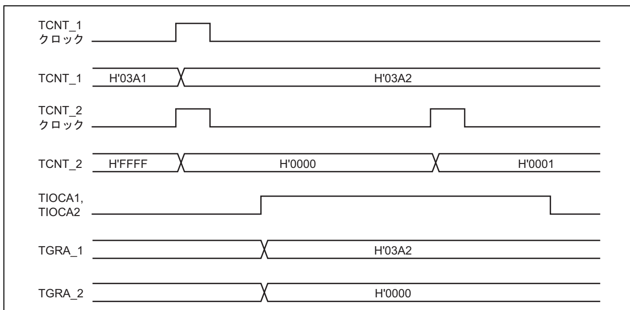
図 9.18 カスケード接続動作例 (1)
