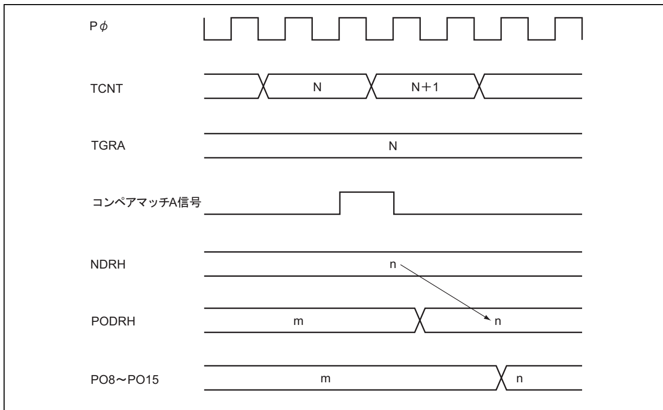
図 10.3 NDR の内容が転送・出力されるタイミング例
