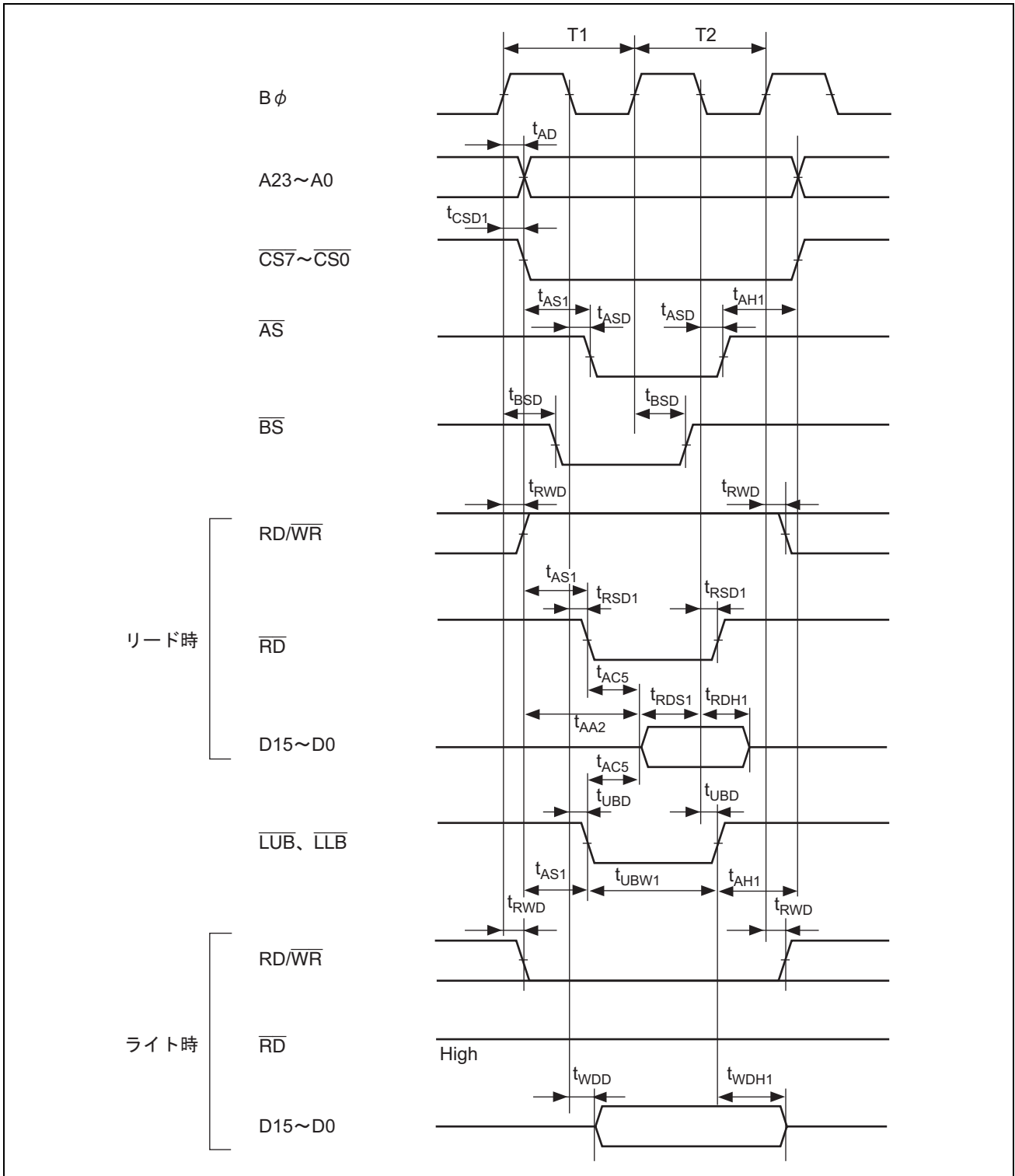
図 20.13 バイト制御 SRAM 2 ステートリード/ライトアクセス
