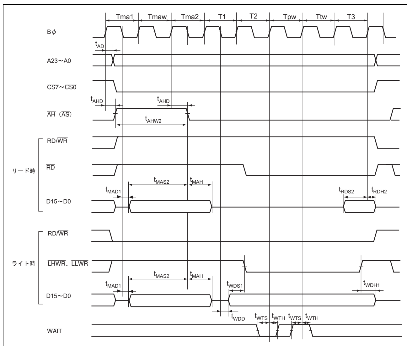
図 20.18 アドレス/データマルチプレクス・アクセスタイミング (ウェイト制御) (-アドレスサイクルプログラムウェイト×1 +データサイクルプログラムウェイト×1+データサイクル端子ウェイト×1の場合)
