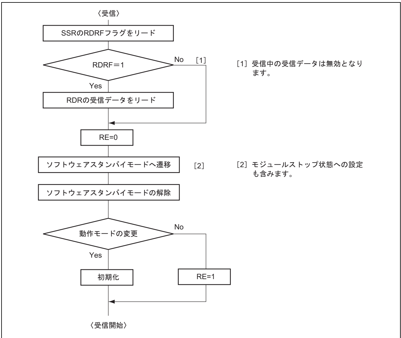
図 13.37 受信時のソフトウェアスタンバイモード遷移フローチャートの例
