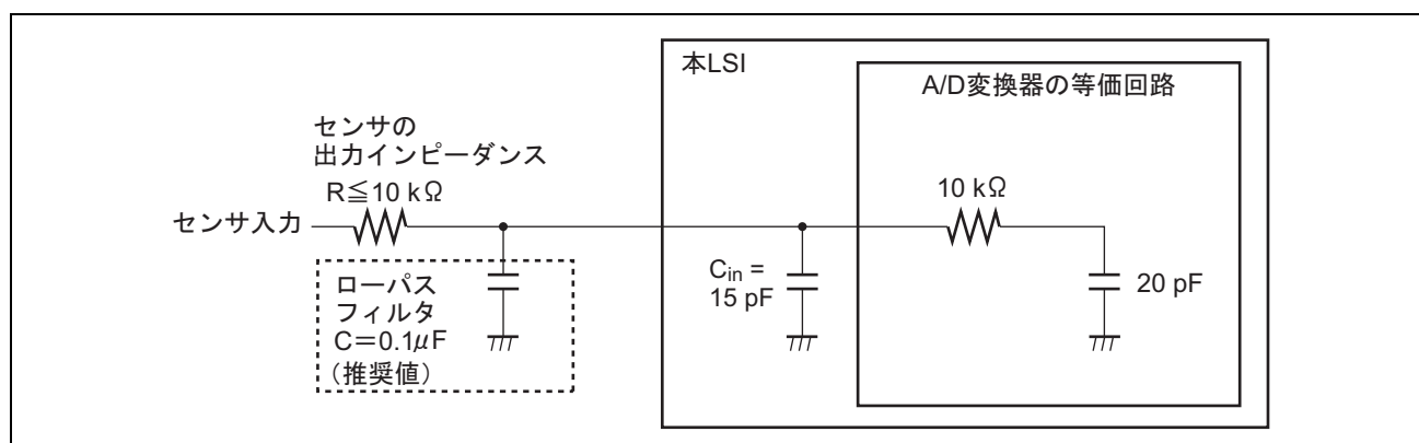
図 14.8 アナログ入力回路の例
