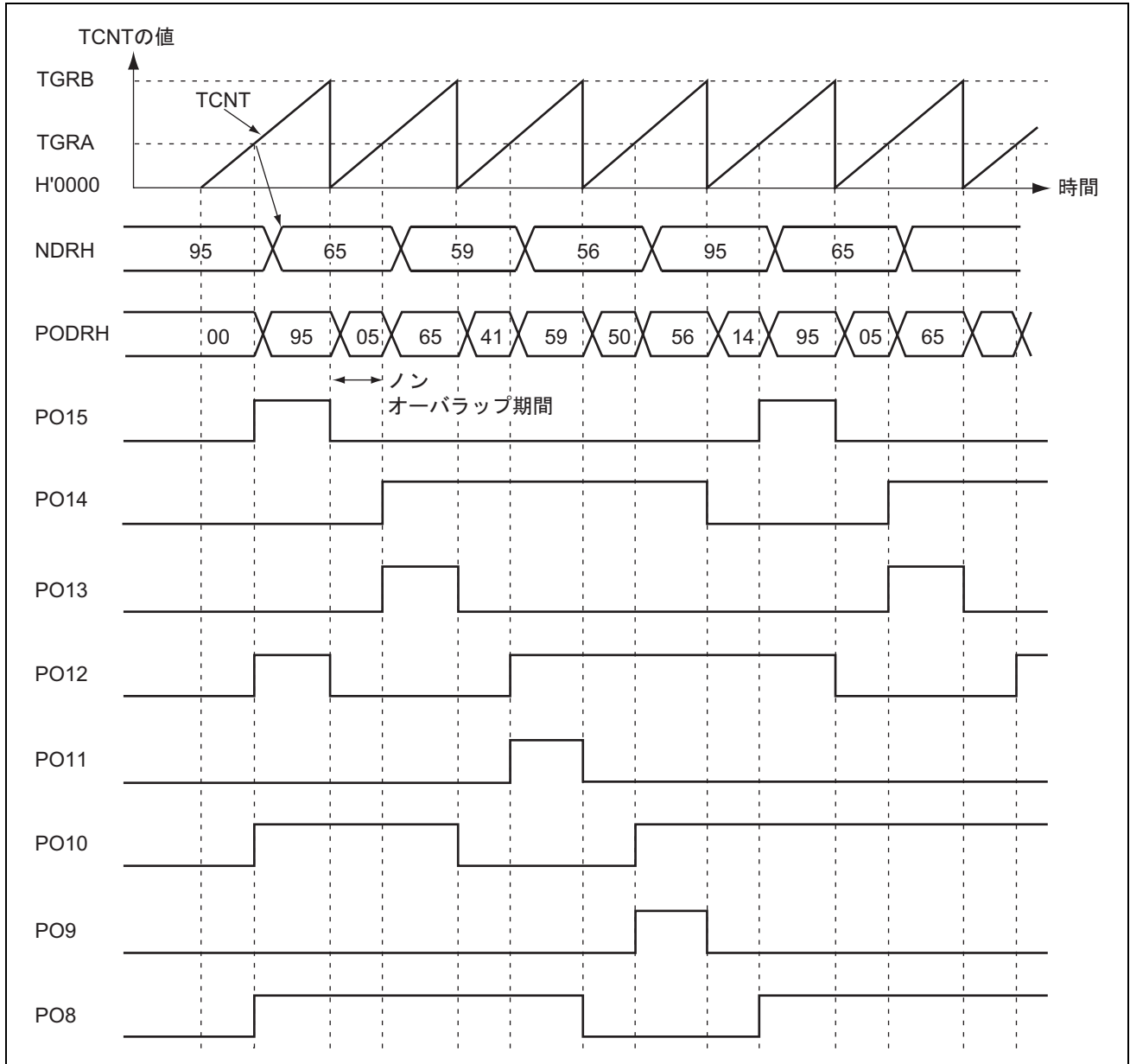
図 10.9 パルス出力ノンオーバーラップ動作例 (4相の相補ノンオーバーラップ出力)
