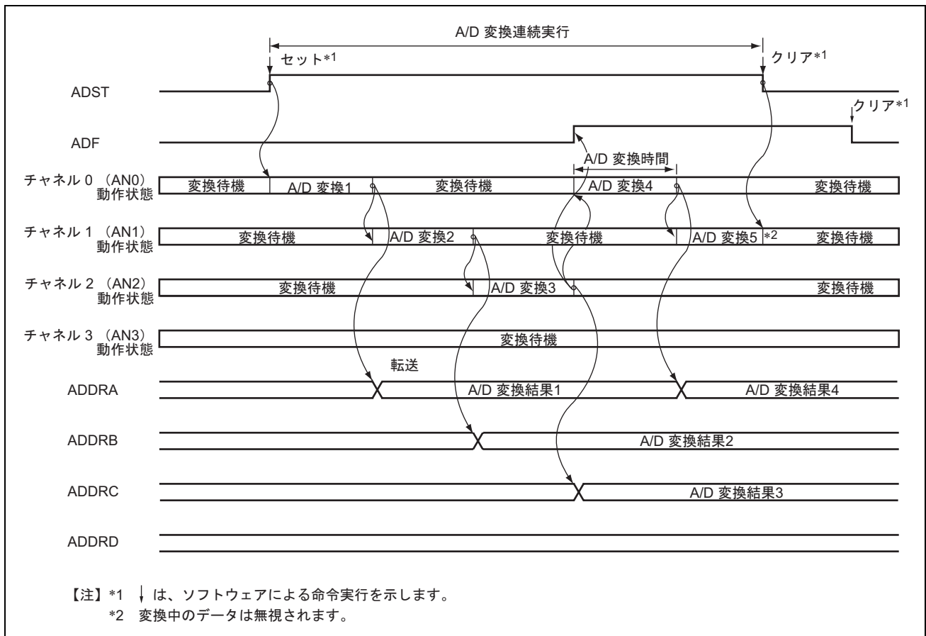
図 14.3 A/D 変換器の動作例（スキャンモード、AN0～AN2 の3チャンネル選択時）
