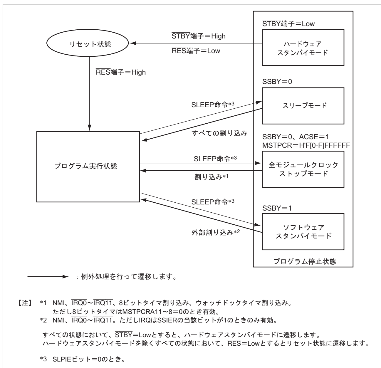
図 18.1 モード遷移図
