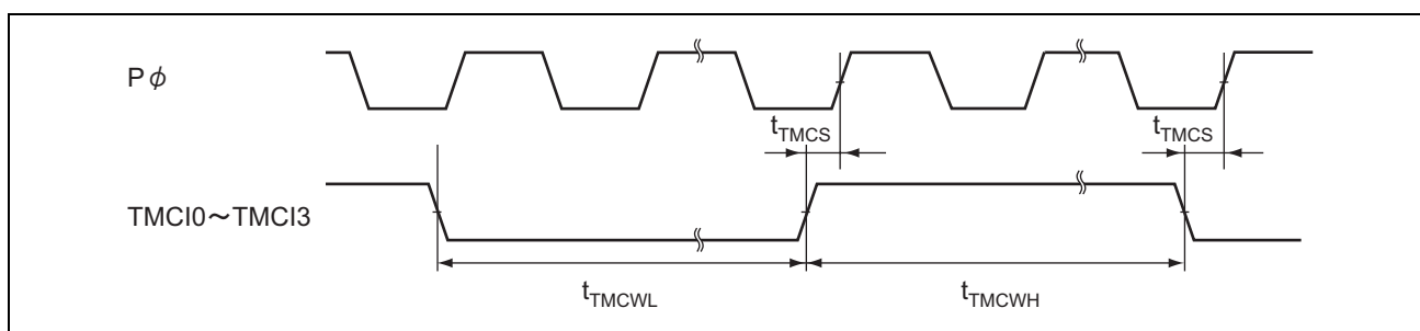
図 20.27 8ビットタイマクロック入力タイミング
