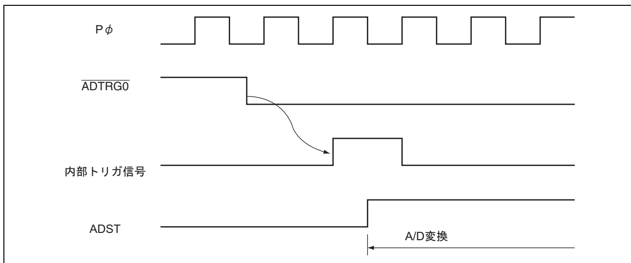
図 14.5 外部トリガ入力タイミング
