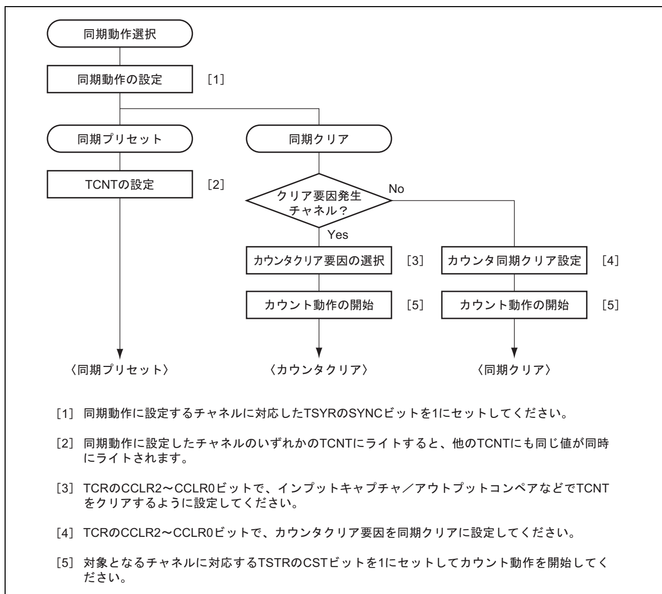
図 9.10 同期動作の設定手順例
