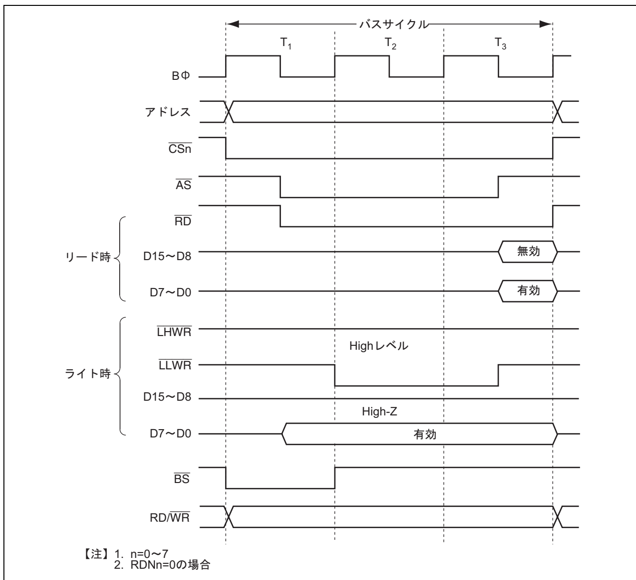
図 6.18 16 ビット 3 ステートアクセス空間のバスタイミング (奇数アドレスバイトアクセス)
