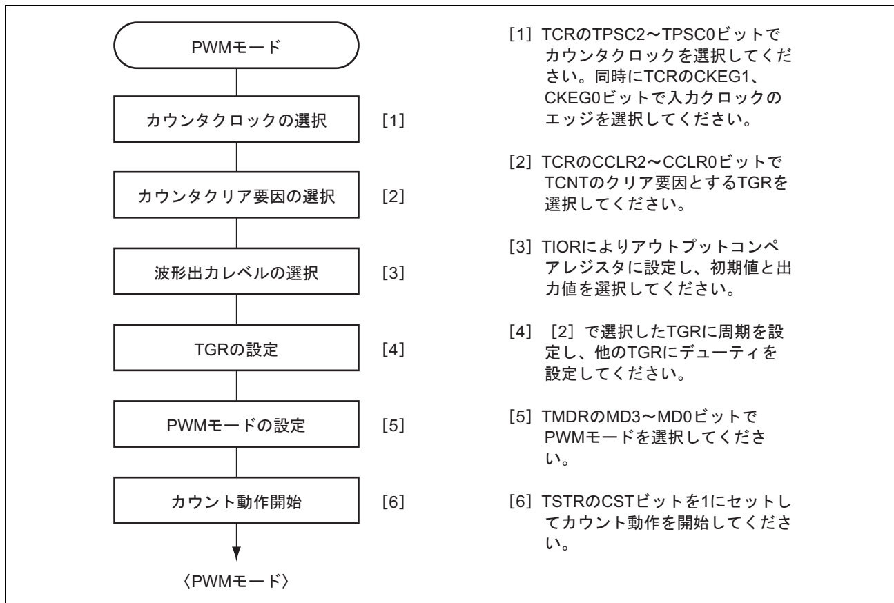
図 9.20 PWM モードの設定手順例
