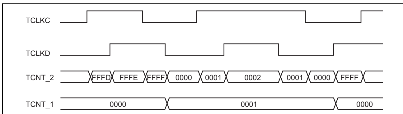
図 9.19 カスケード接続動作例 (2)
