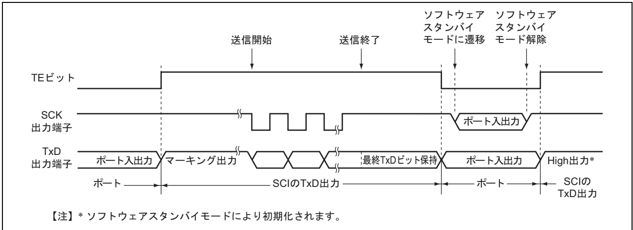
図 13.36 ソフトウェアスタンバイモード遷移時のポートの端子状態（内部クロック、クロック同期送信）
