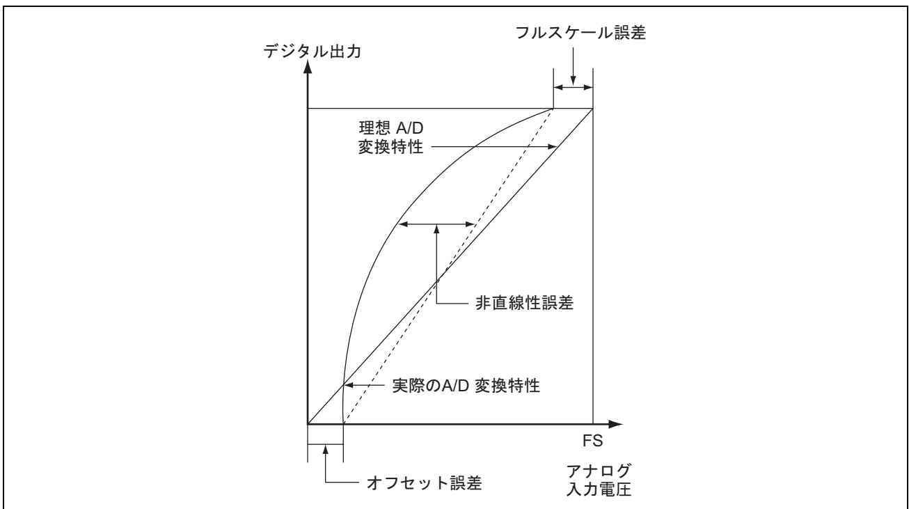
図 14.7 A/D 変換精度の定義
