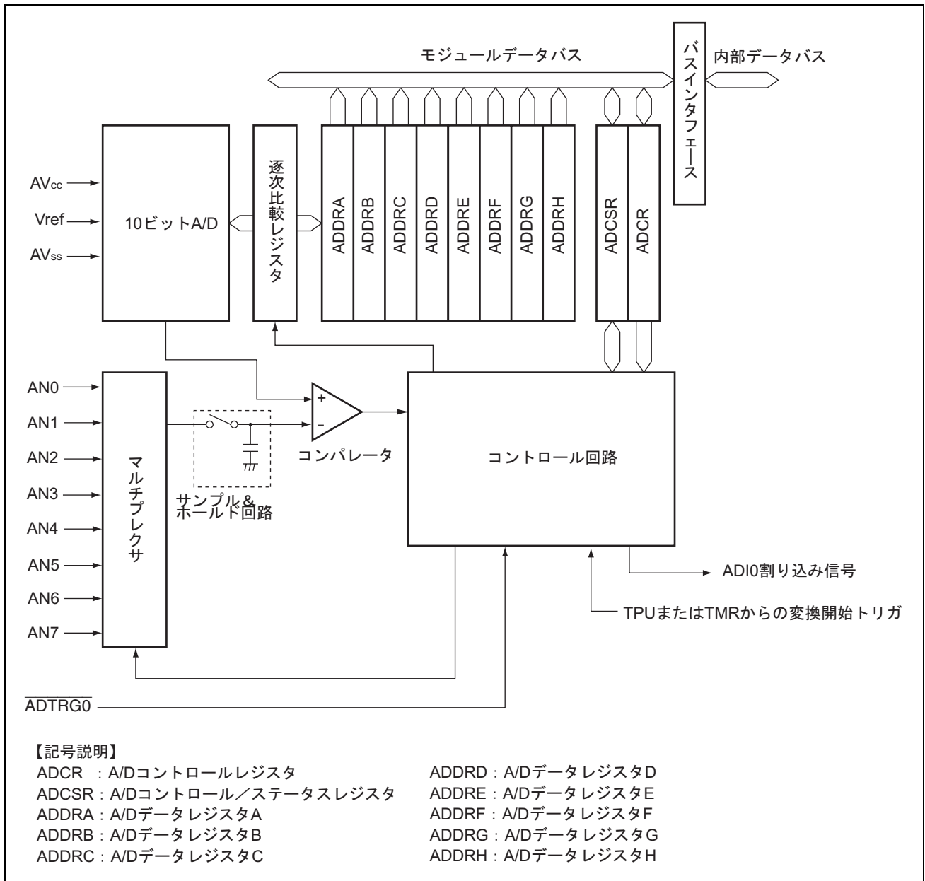
図 14.1 A/D 変換器のブロック図
