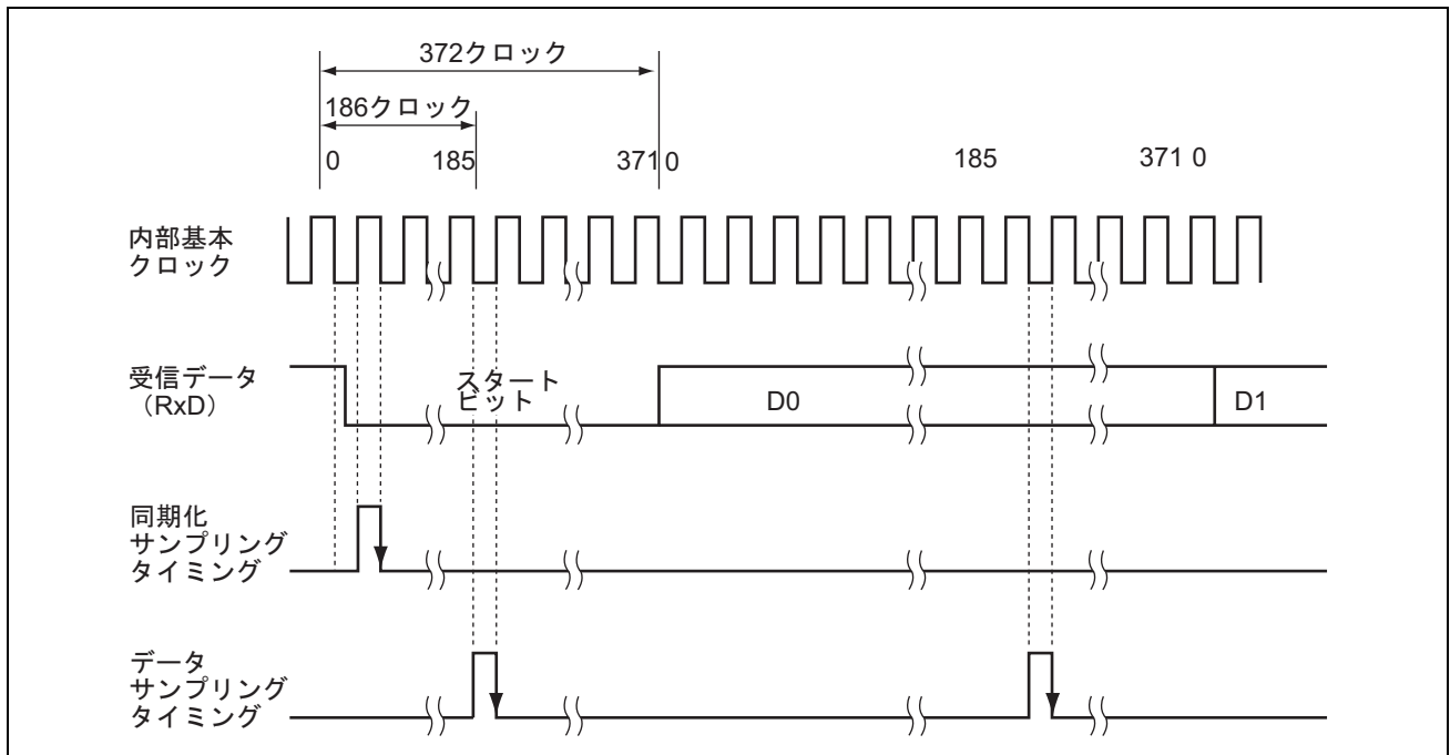
図 13.25 スマートカードインタフェースモード時の受信データサンプリングタイミング (372倍のクロック使用時)
