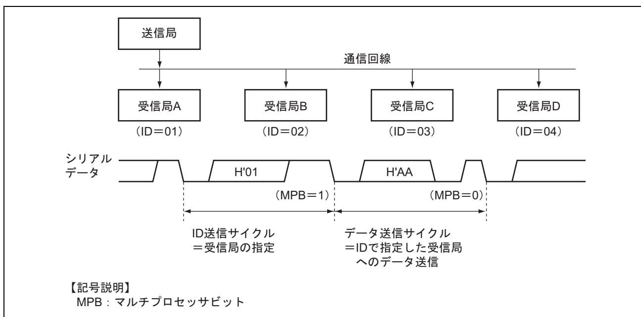
図 13.10 マルチプロセッサフォーマットを使用した通信例（受信局 A へのデータ H'AA の送信の例）
