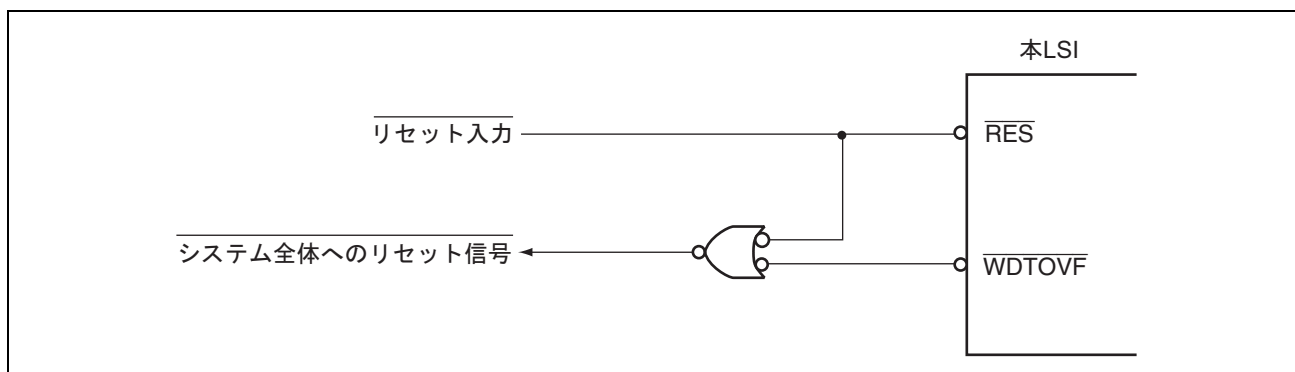
図 12.6 \overline{\text{WDTOVF}} 信号によるシステムのリセット回路例
