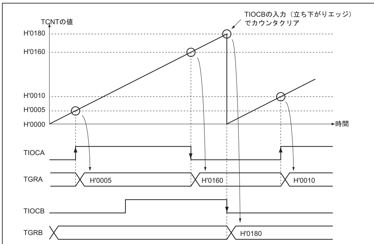
図 9.9 インพุットキャプチャ動作例
