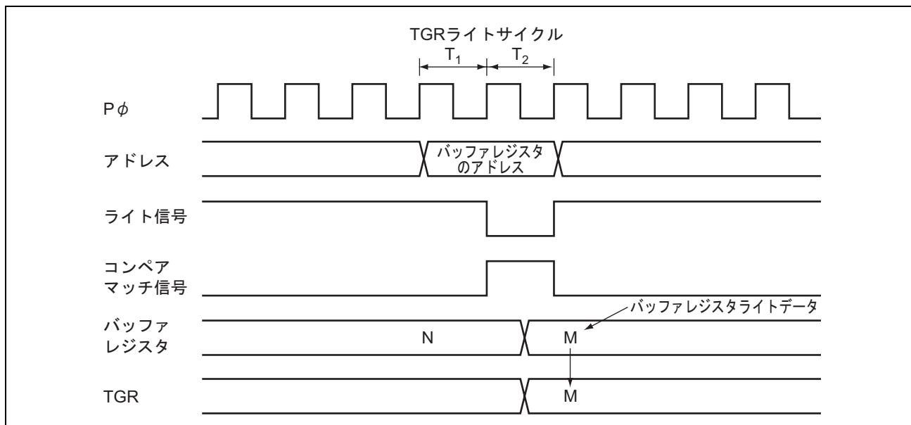
図 9.49 バッファレジスタのライトとコンペアマッチの競合
