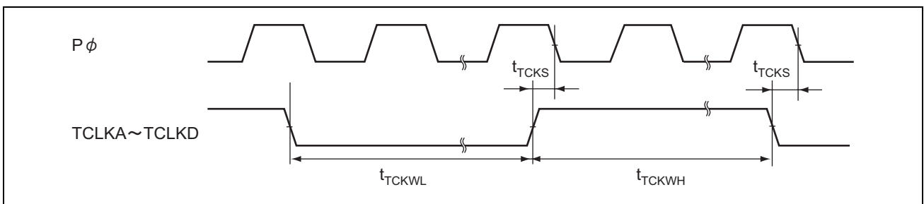
図 20.23 TPU クロック入力タイミング
