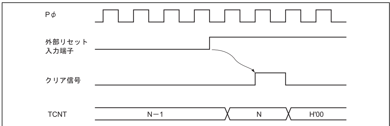
図 11.10 外部リセット入力によるクリアタイミング (立ち上がりエッジ)
