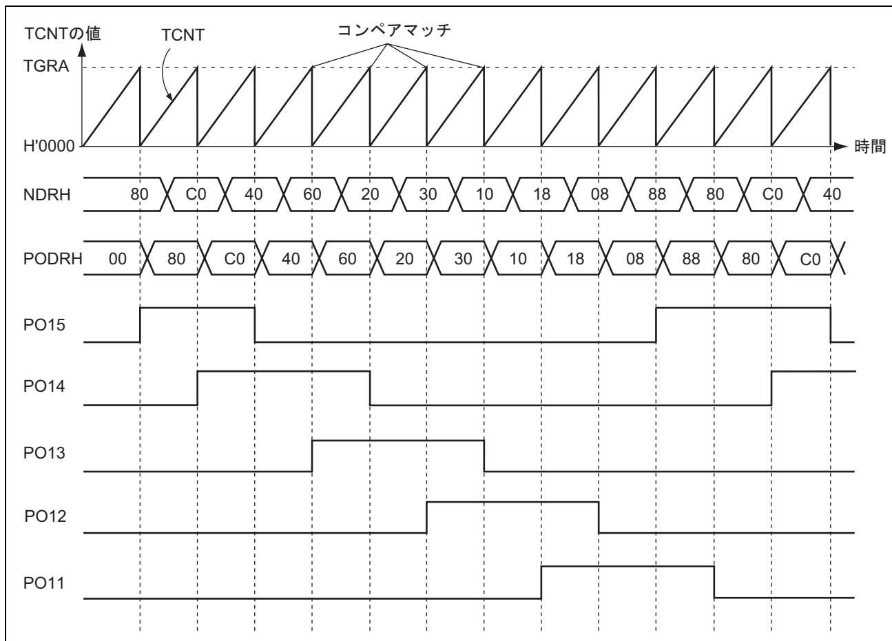
図 10.5 パルス出力通常動作例 (5相パルス出力例)
