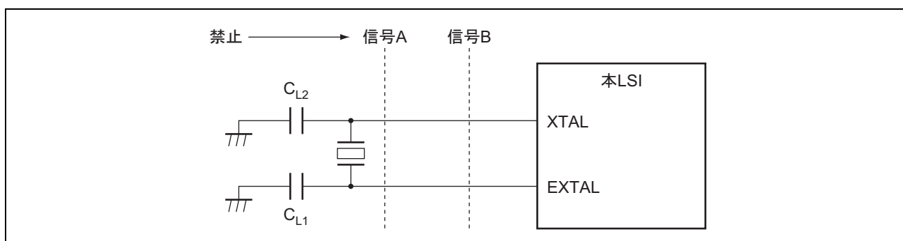
図 17.6 発振回路部のボード設計に関する注意事項
