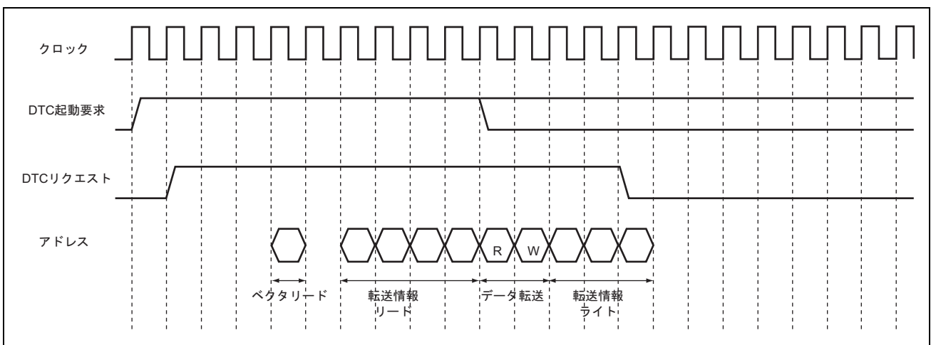
図 7.14 DTC の動作タイミング例 (フルアドレスモード、ノーマル転送モード、リピート転送モード)
