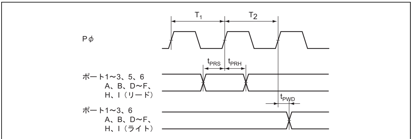
図 20.21 I/O ポート入出力タイミング
