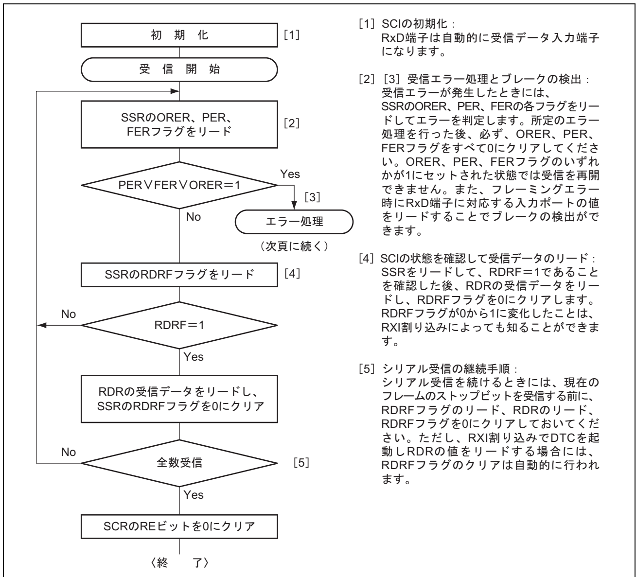
図 13.9 シリアル受信のフローチャートの例 (1)
