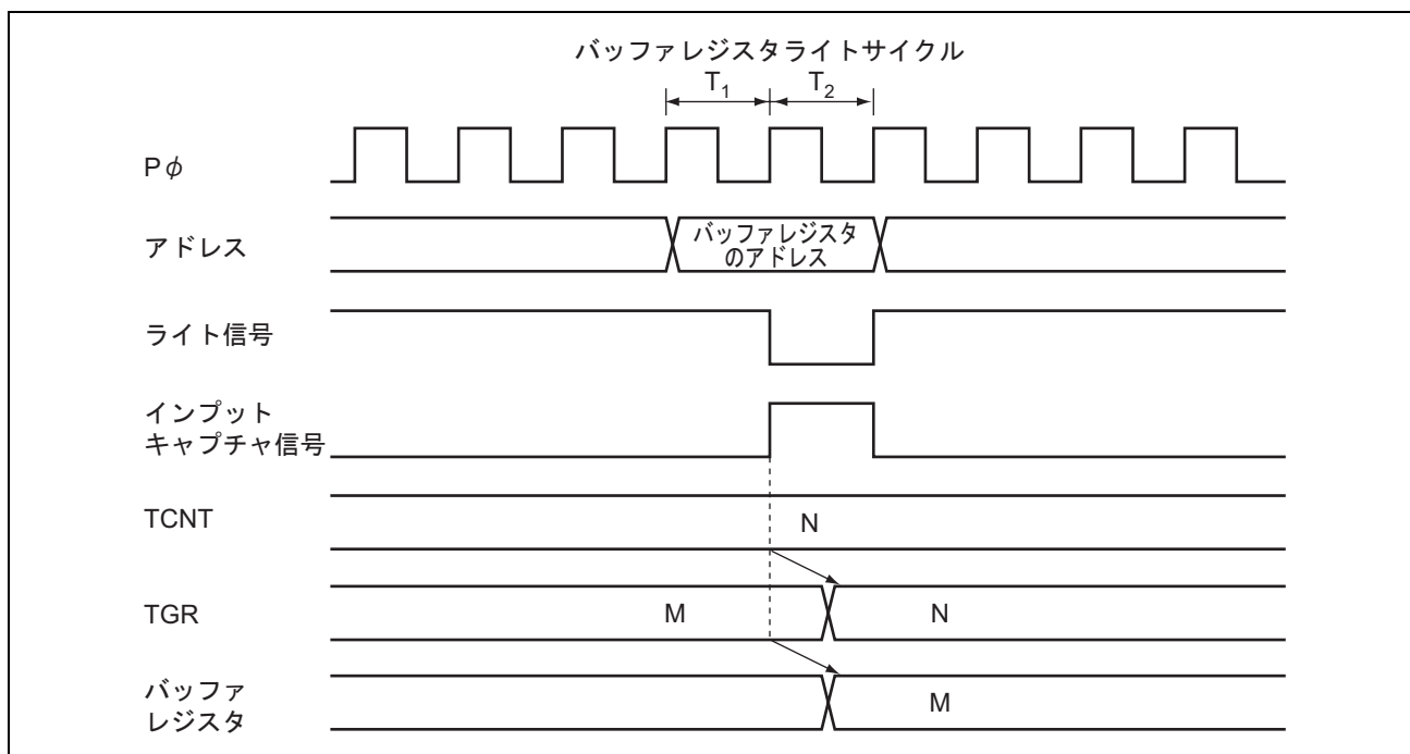
図 9.52 バッファレジスタのライトと入力キャプチャの競合
