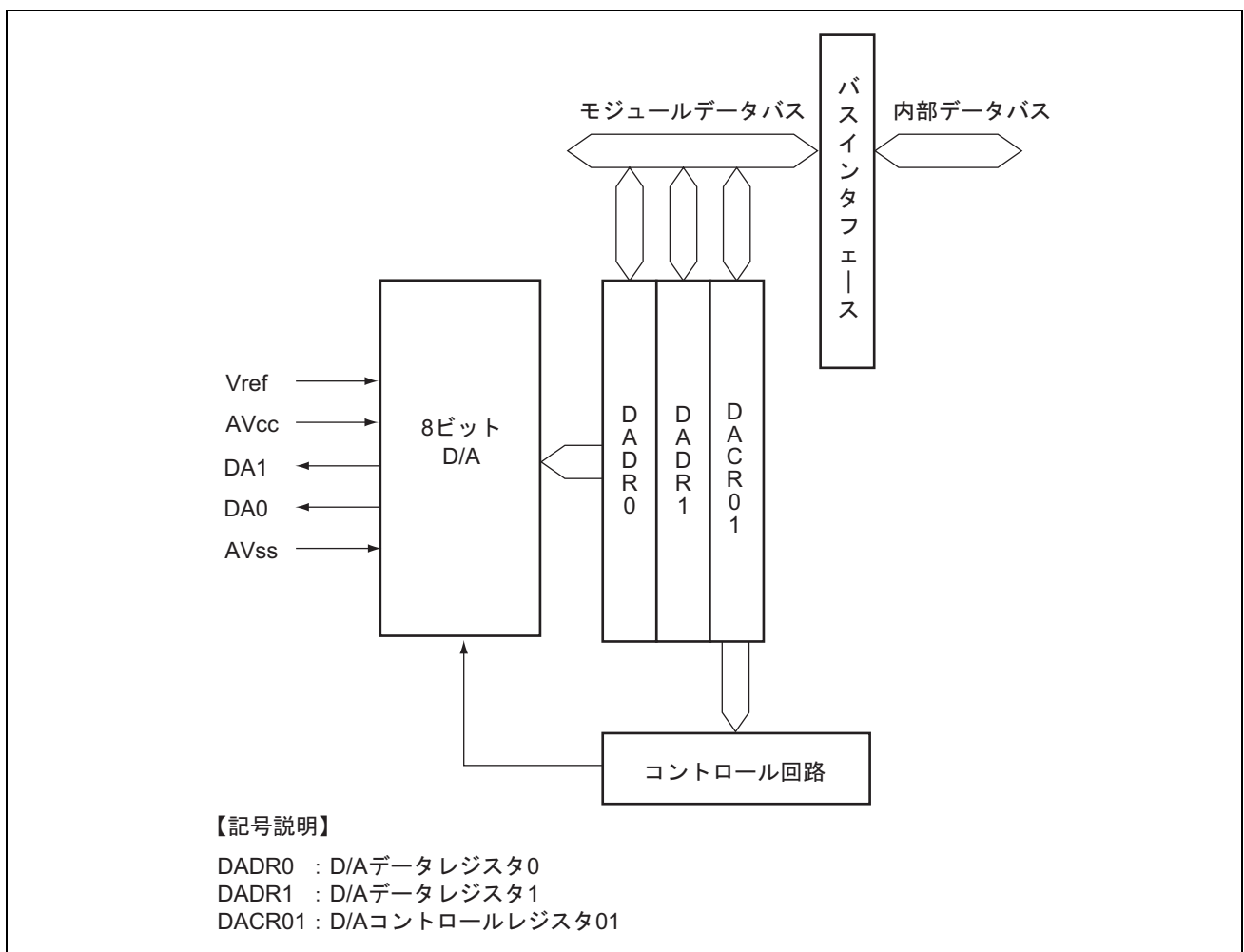
図 15.1 D/A 変換器のブロック図
