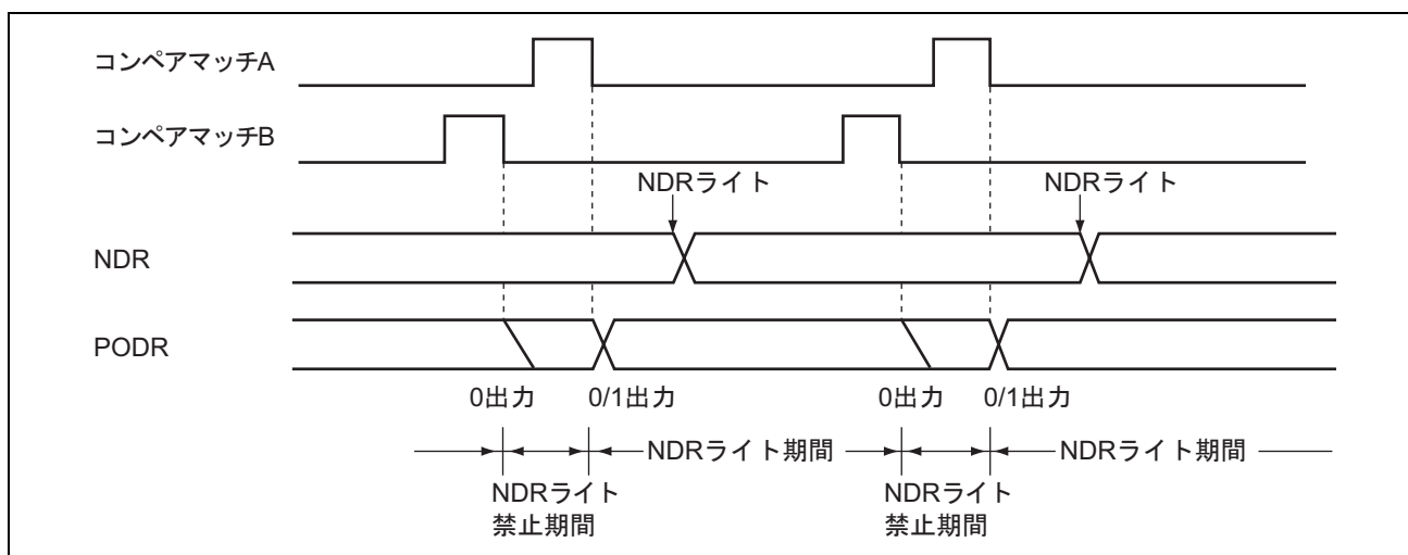
図 10.7 ノンオーバーラップ動作と NDR ライトタイミング
