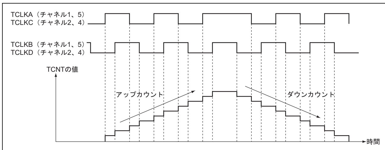
図 9.25 位相計数モード 1 の動作例
