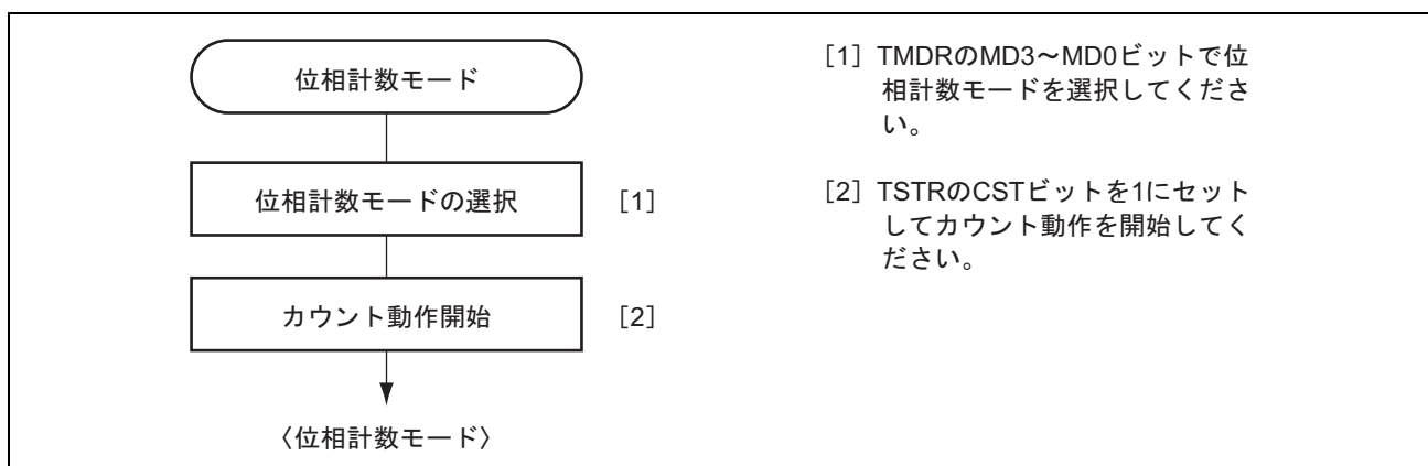
図 9.24 位相計数モードの設定手順例
