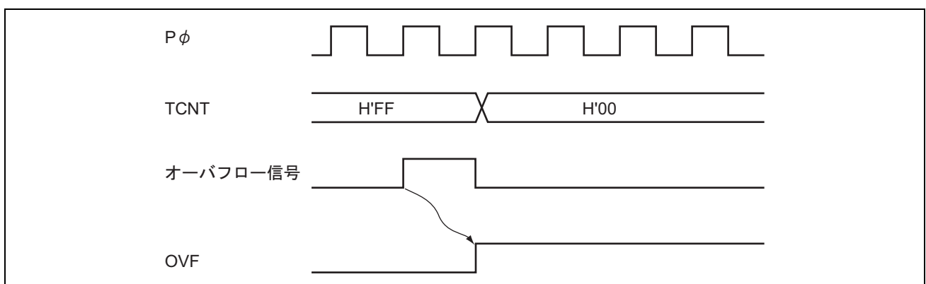
図 11.12 OVF フラグのセットタイミング
