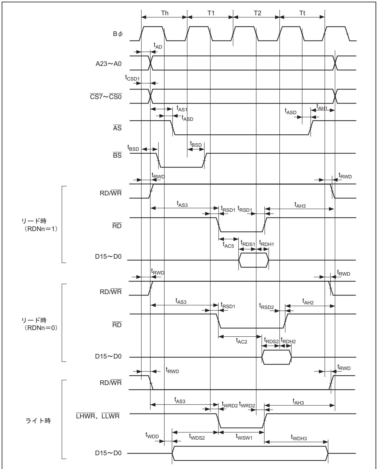
図 20.11 基本バスタイミング/2 ステートアクセス (CS アサート期間延長)
