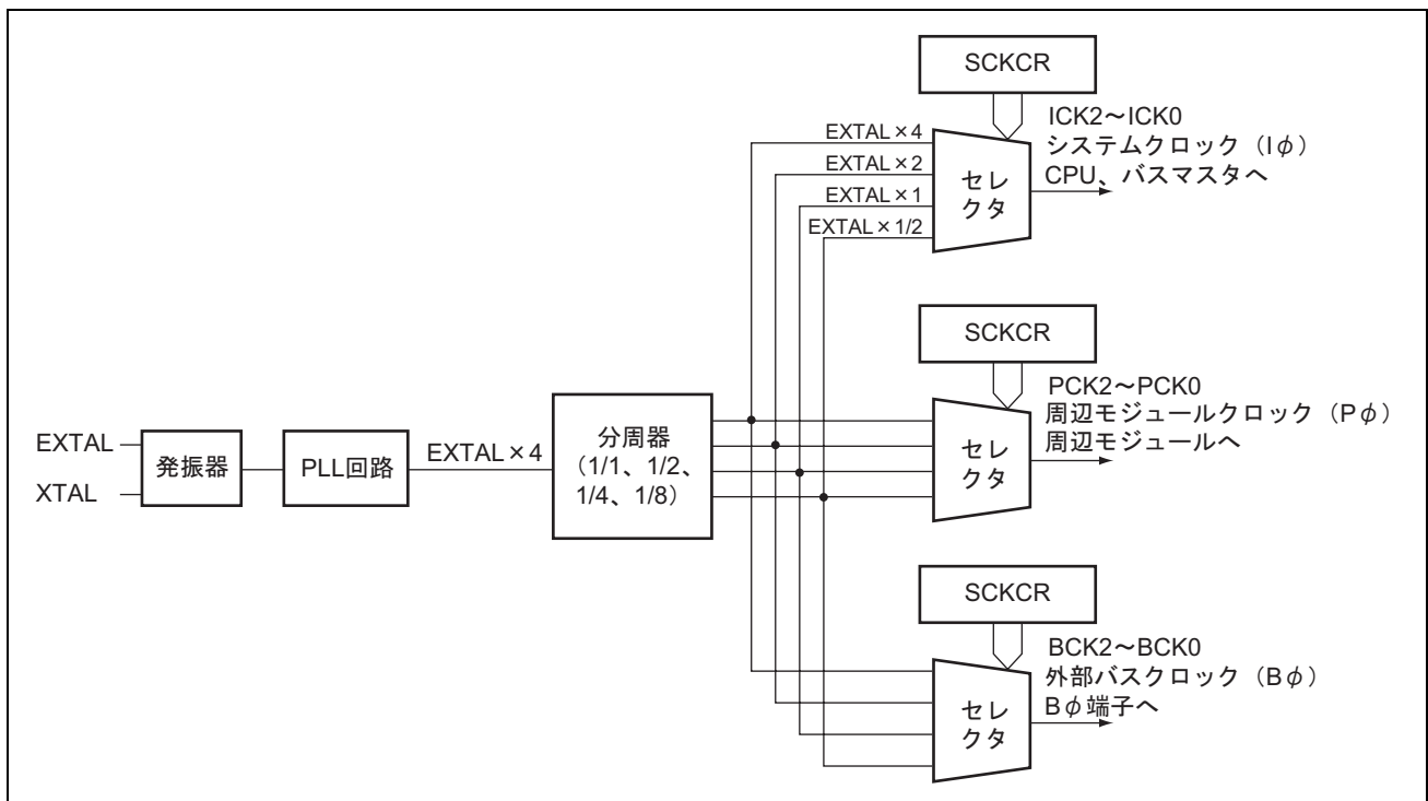
図 17.1 クロック発振器のブロック図
