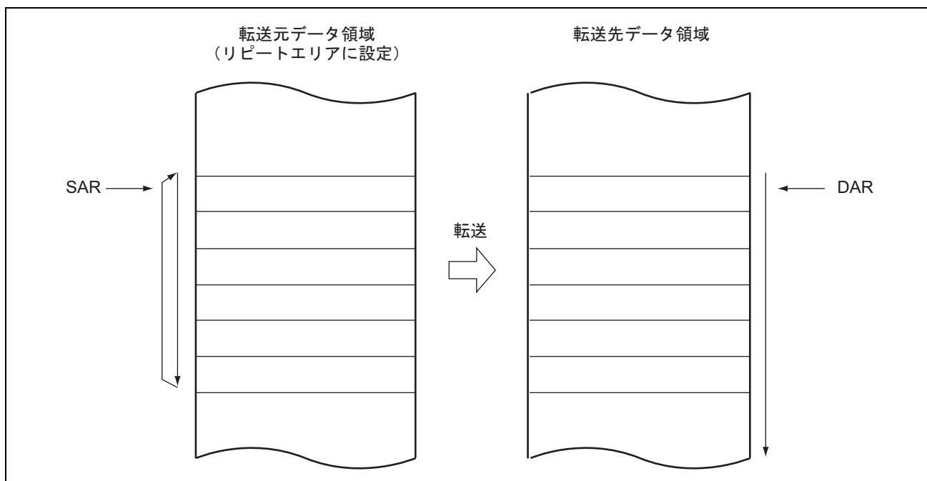
図 7.8 リピート転送モードのメモリマップ (転送元をリピートエリアに指定した場合)
