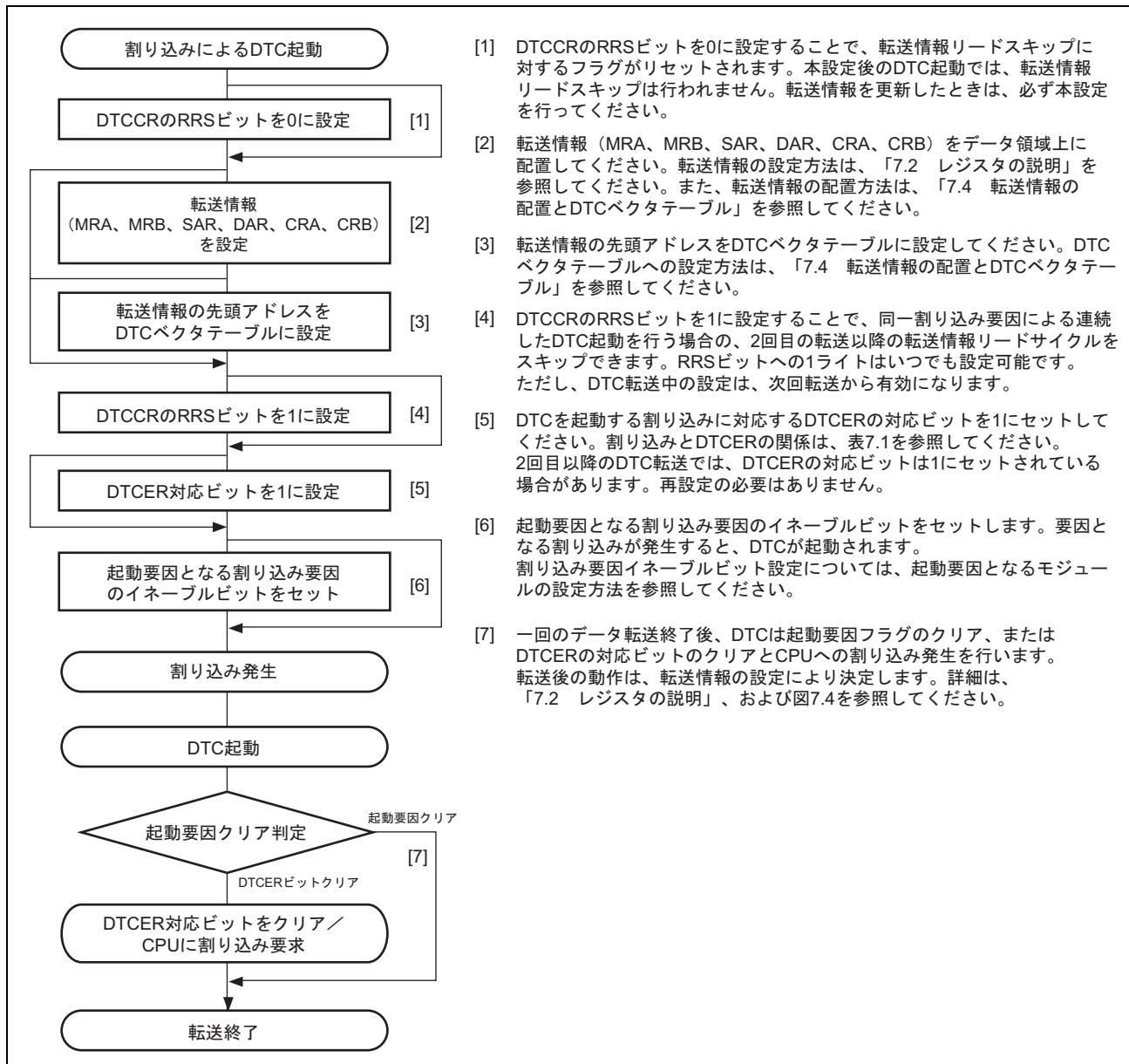
図 7.15 割り込みによる DTC 起動方法
