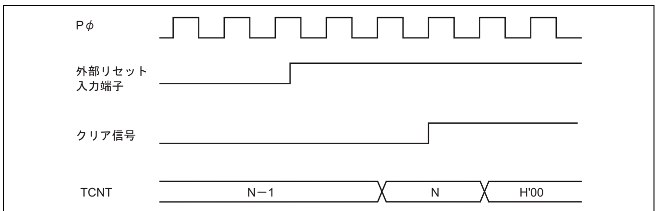
図 11.11 外部リセット入力によるクリアタイミング (ハイレベル)
