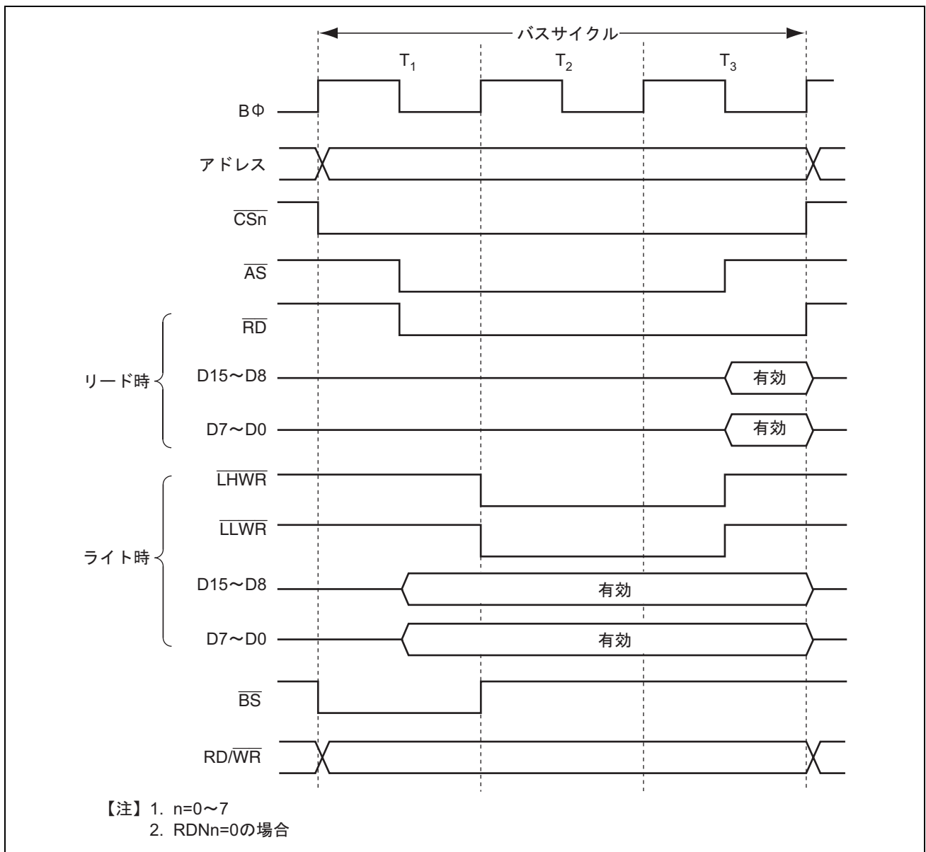
図 6.19 16 ビット 3 ステートアクセス空間のバスタイミング (偶数アドレスワードアクセス)
