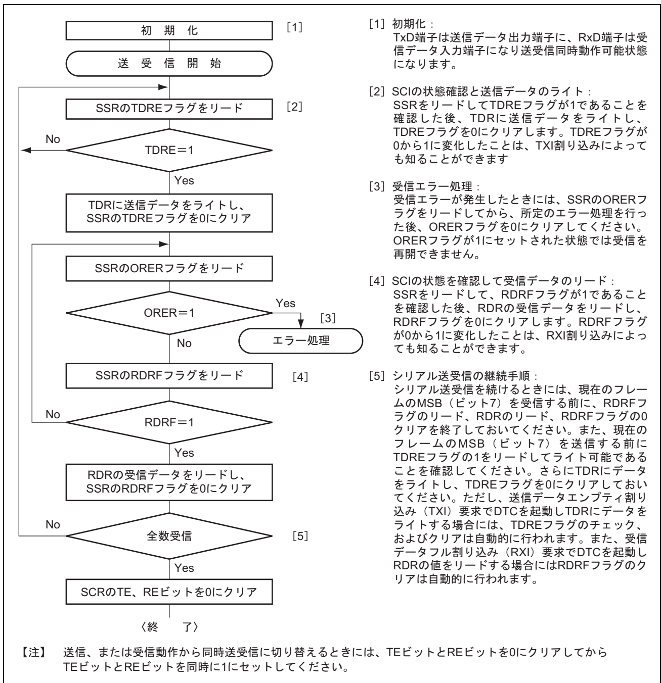
図 13.20 シリアル送受信同時動作のフローチャートの例
