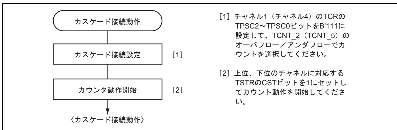
図 9.17 カスケード接続動作設定手順例
