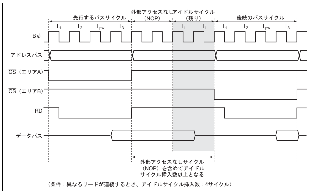
図 6.37 アイドルサイクル挿入例
