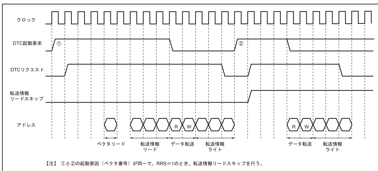
図 7.6 転送情報リードスキップのタイミングチャート
