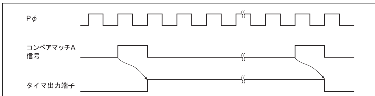
図 11.8 コンペアマッチ A 信号によるトグル出力のタイマ出力タイミング
