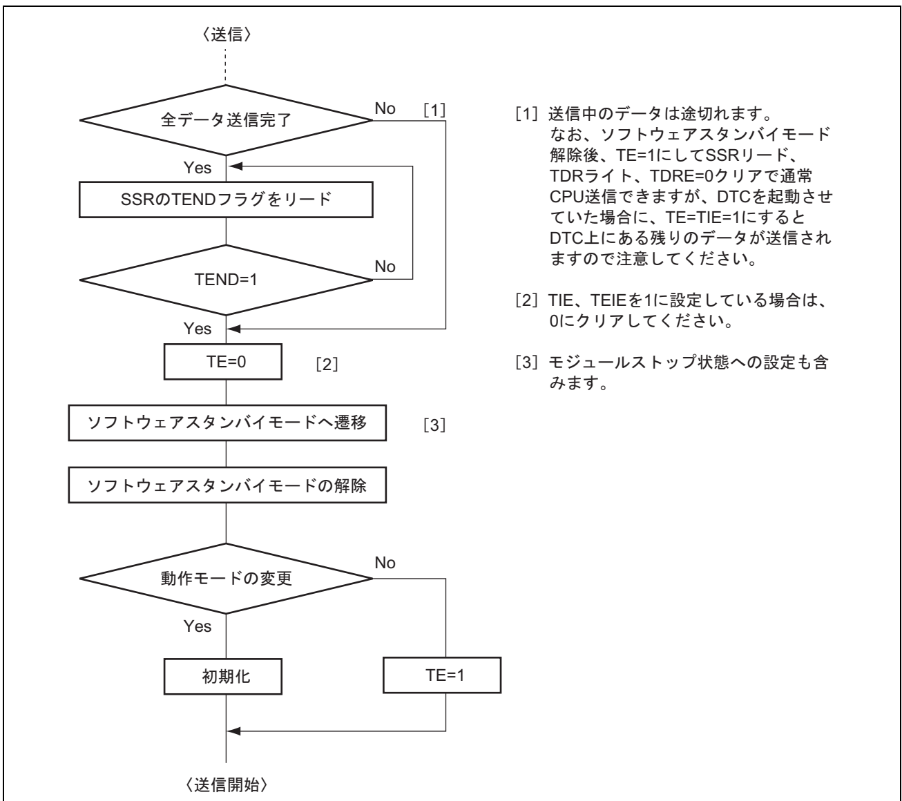
図 13.34 送信時のソフトウェアスタンバイモード遷移フローチャートの例
