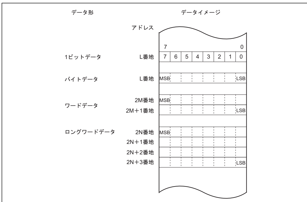
図 2.13 メモリ上でのデータ形式
