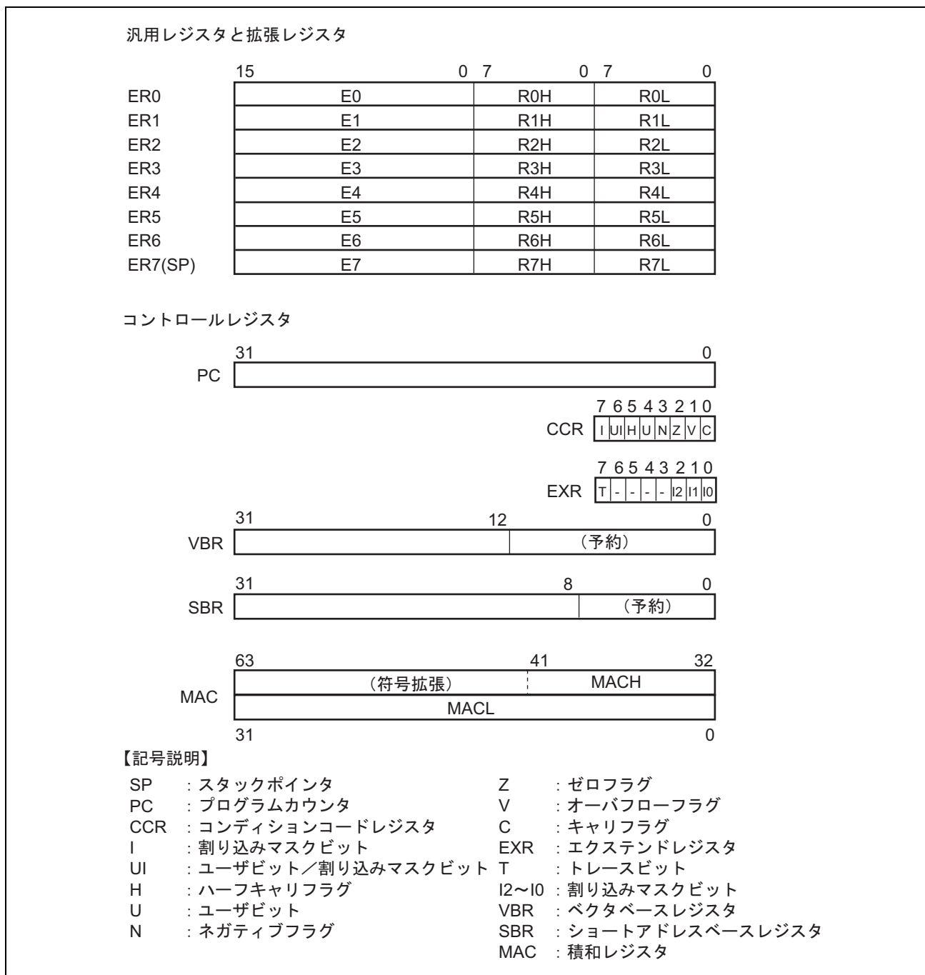
図 2.9 CPU 内部レジスタ構成
