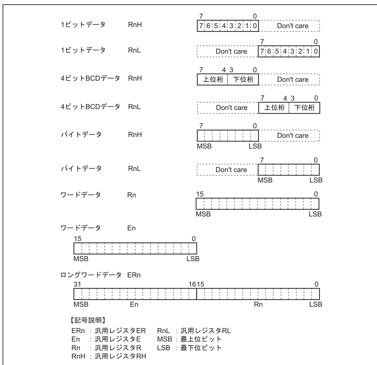
図 2.12 汎用レジスタのデータ形式
