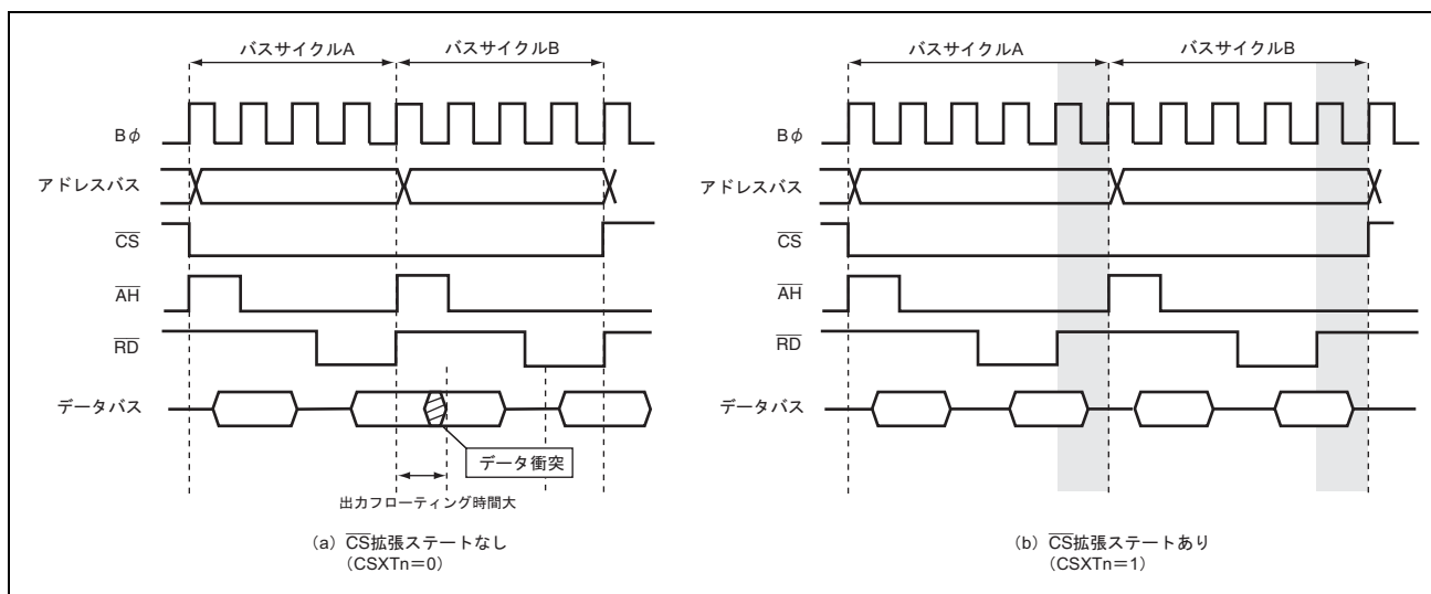
図 6.33 同一エリアのアドレス/データマルチプレクス I/O 空間連続リード
