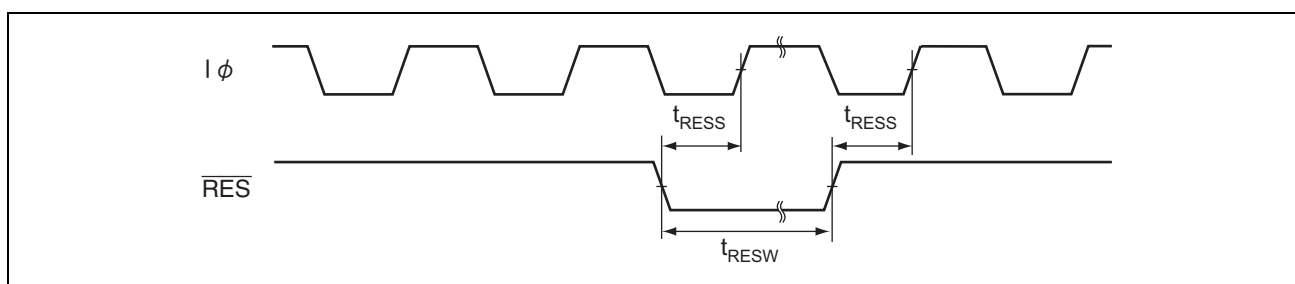
図 20.6 リセット入力タイミング
