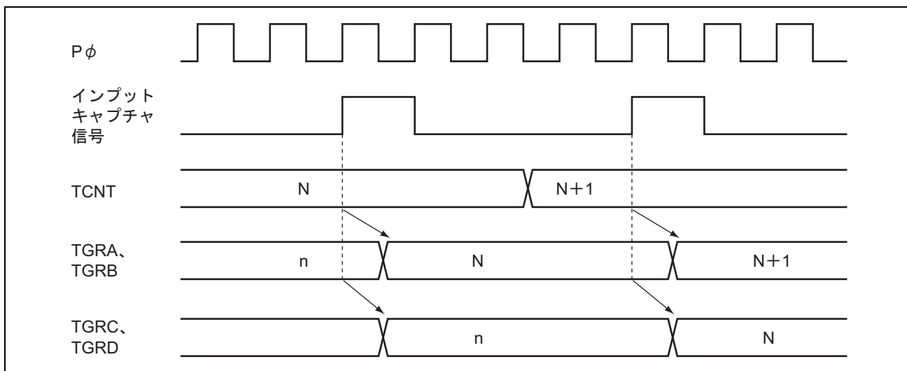
図 9.37 バッファ動作タイミング (入力キャプチャ)
