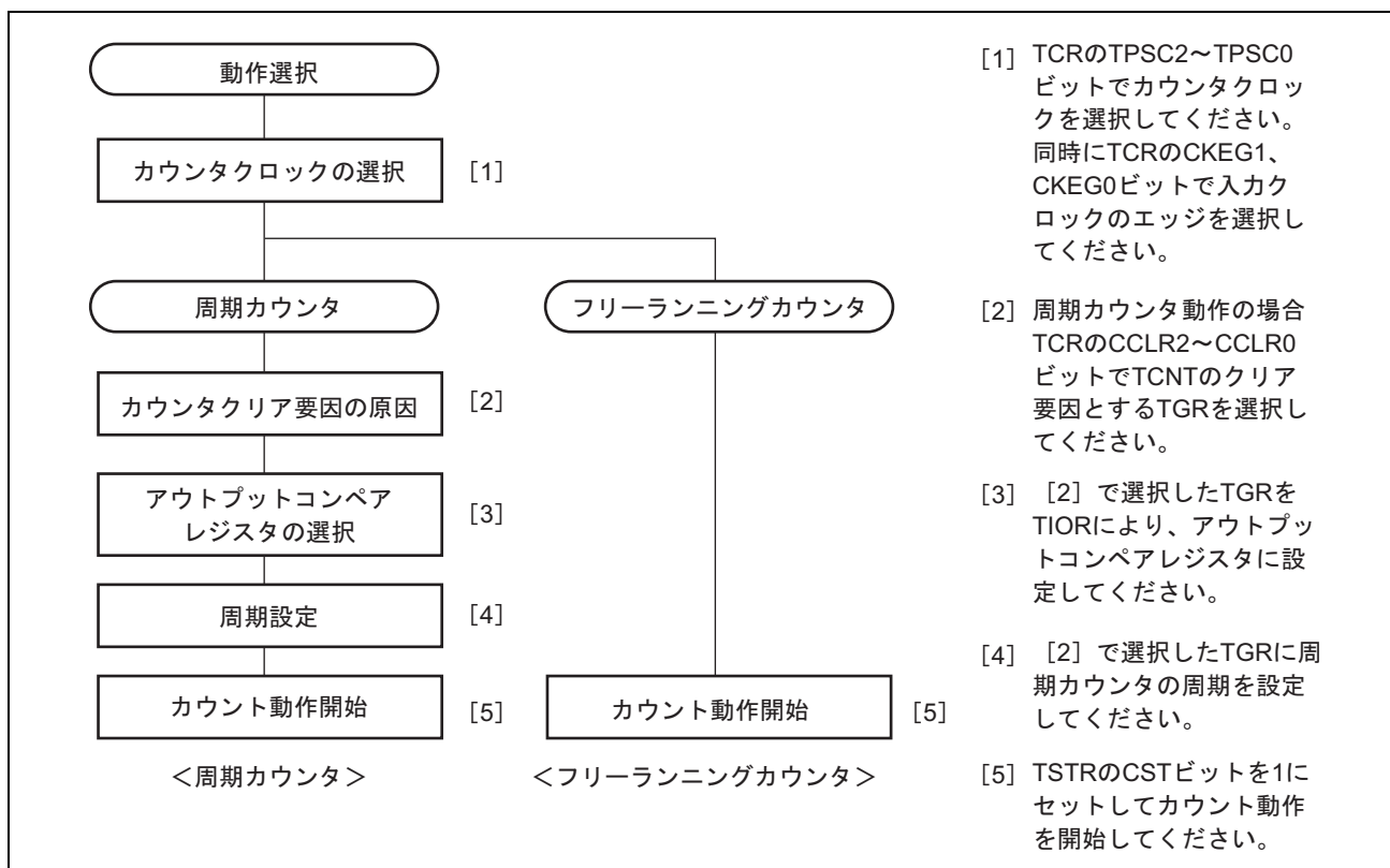
図 9.2 カウンタ動作設定手順例
