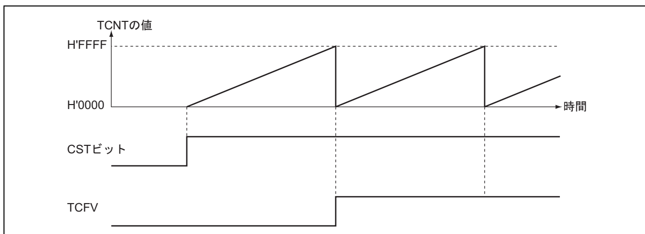
図 9.3 フリーランニングカウンタの動作
