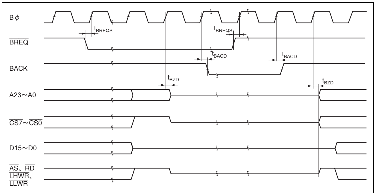
図 20.19 外部バス権開放タイミング
