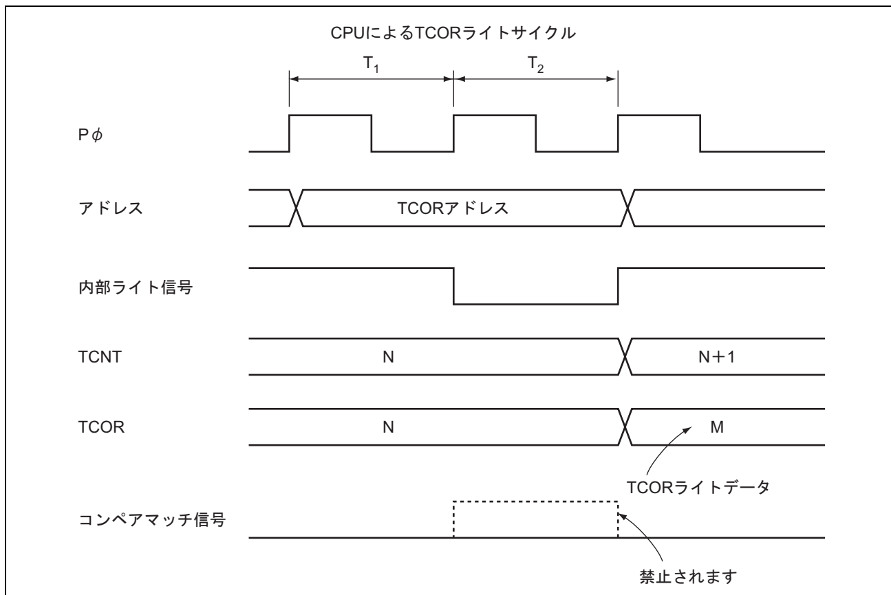
図 11.15 TCOR のライトとコンペアマッチの競合
