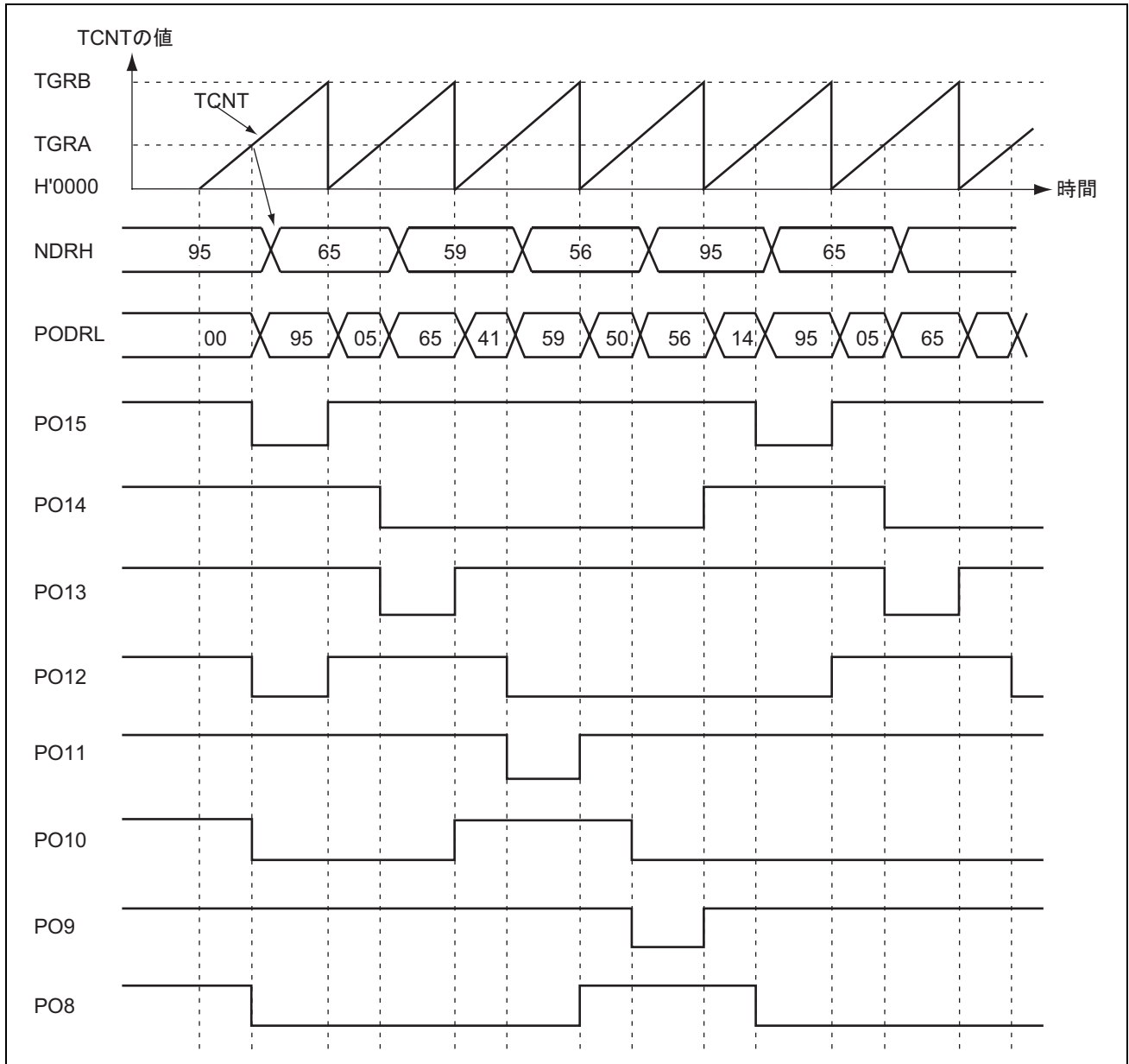
図 10.10 パルス反転出力例
