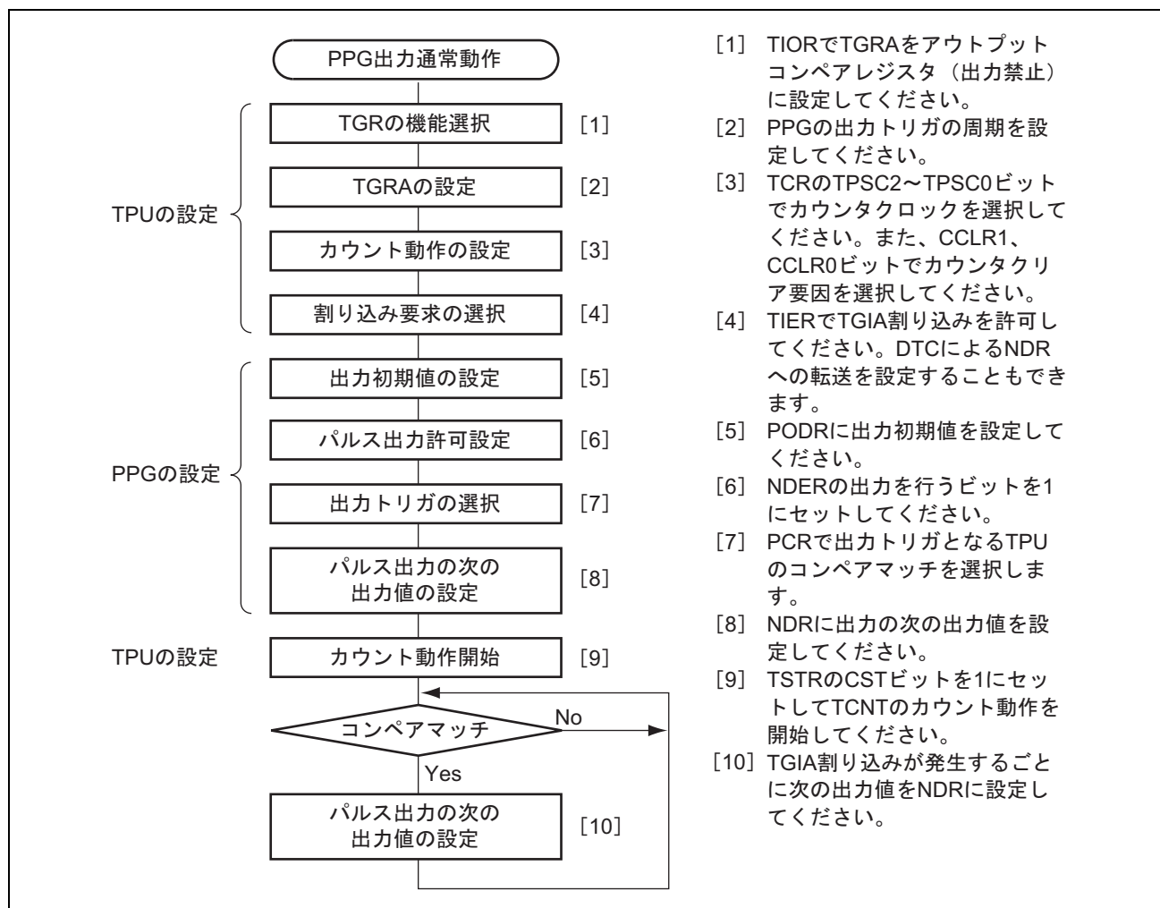
図 10.4 パルス出力通常動作の設定手順例
