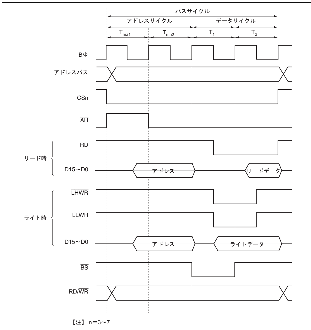
図 6.29 16 ビットアクセス空間へのアクセスタイミング (ABWHn=0、ABWLn=1)
