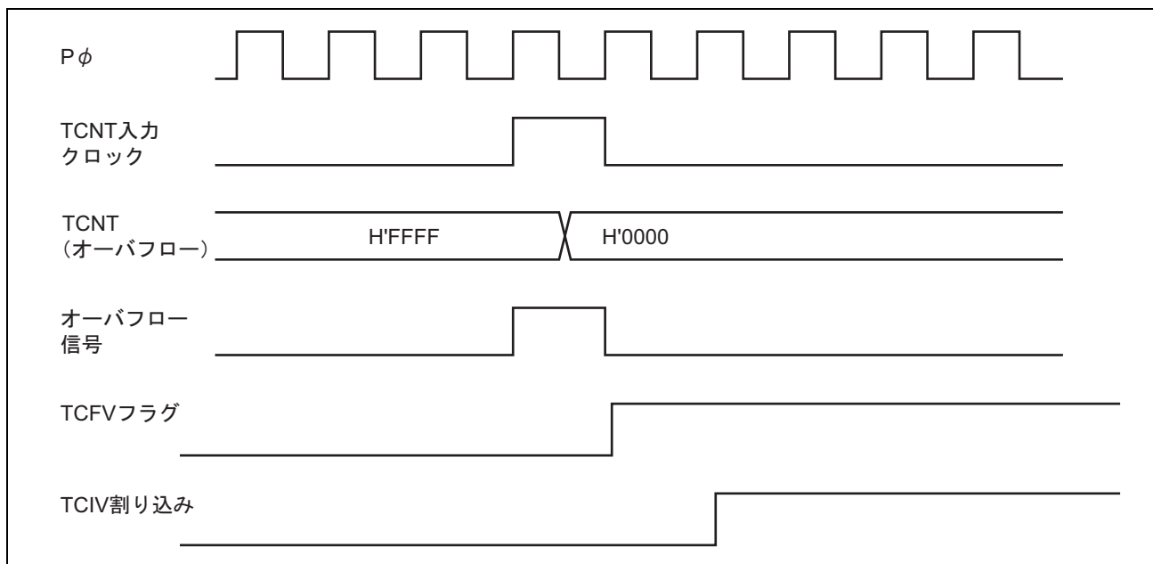
図 9.40 TCIV 割り込みのセットタイミング
