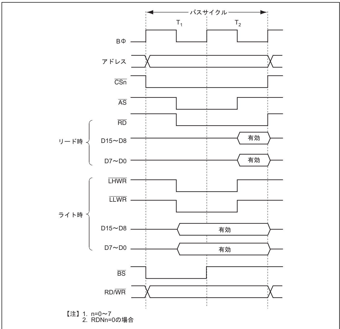
図 6.16 16 ビット 2 ステートアクセス空間のバスタイミング (偶数アドレスワードアクセス)
