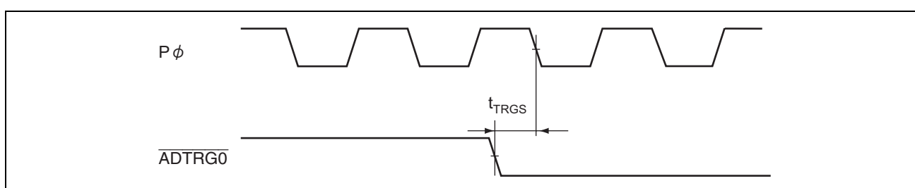
図 20.31 A/D 変換器外部トリガ入力タイミング
