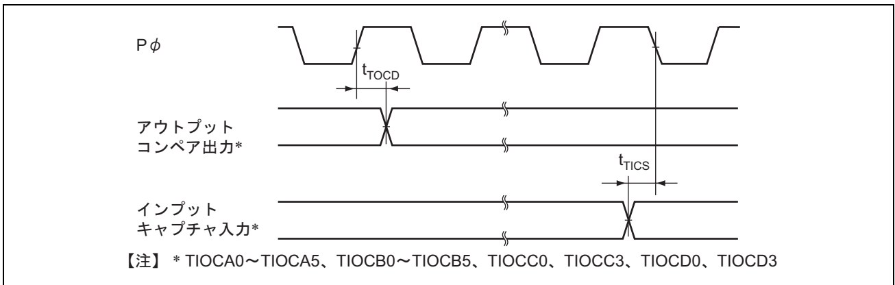
図 20.22 TPU 入出力タイミング
