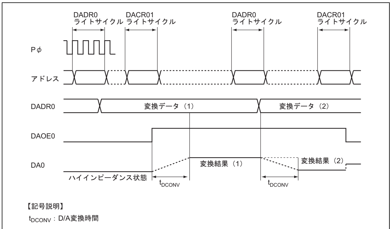
図 15.2 D/A 変換器の動作例
