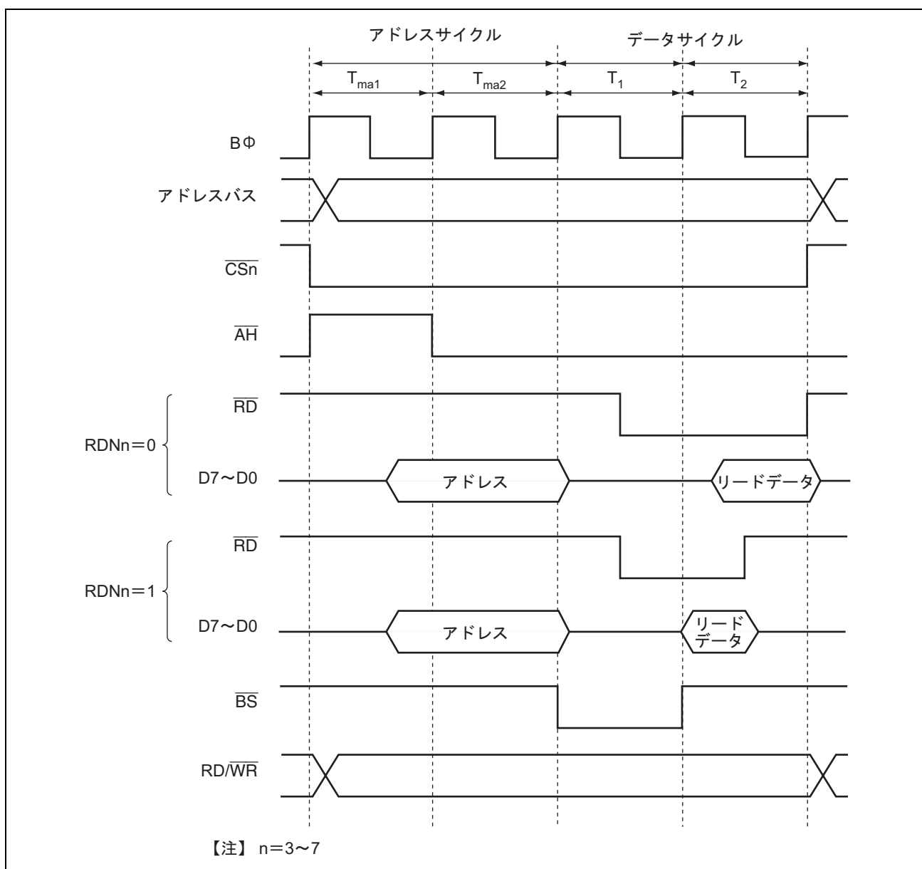
図 6.31 リードストロークタイミング例
