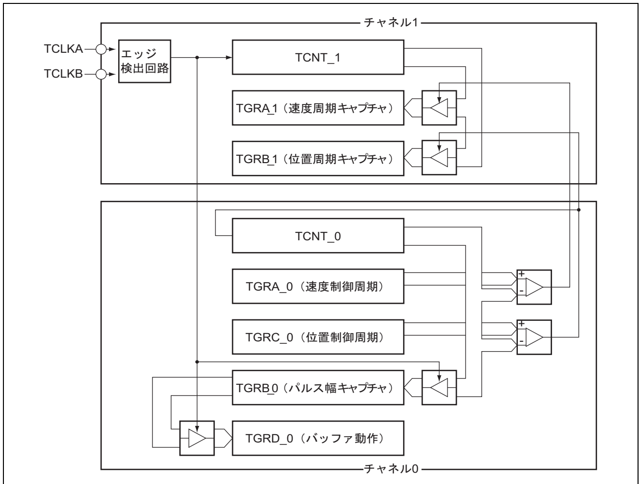
図 9.29 位相計数モードの応用例
