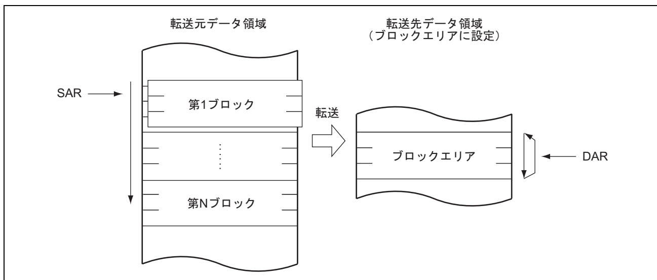
図 7.9 ブロック転送モードのメモリマップ (転送先をブロックエリアに指定した場合)
