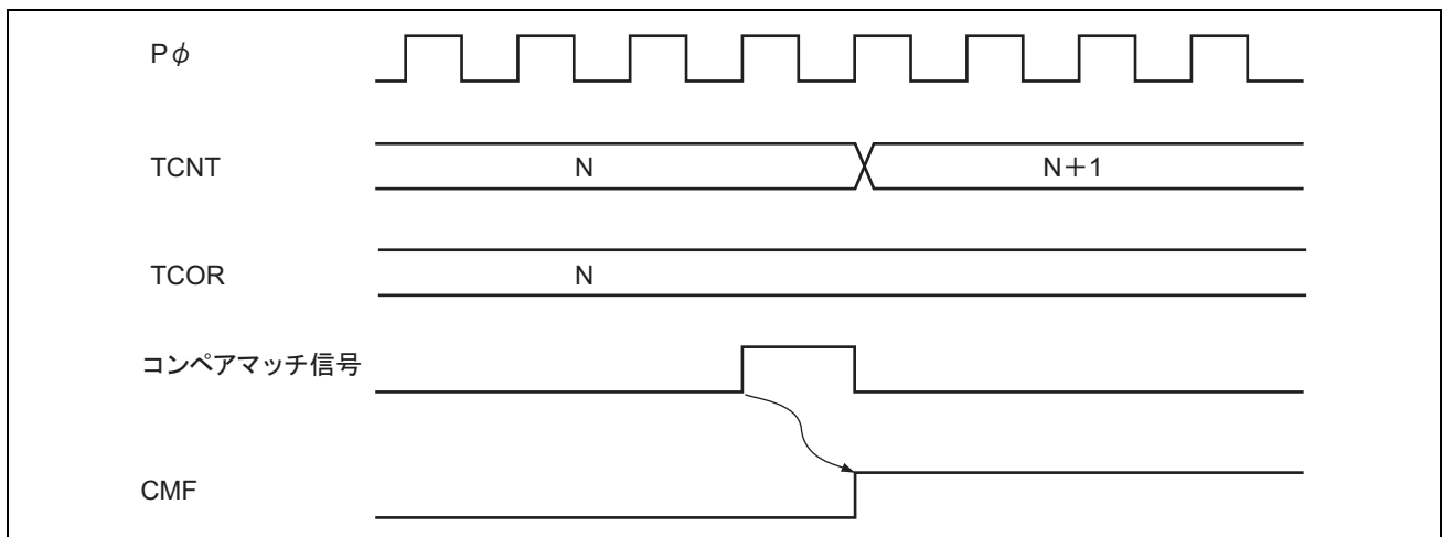
図 11.7 コンペアマッチ時の CMF フラグのセットタイミング
