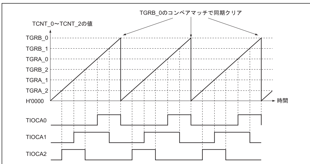
図 9.11 同期動作の動作例
