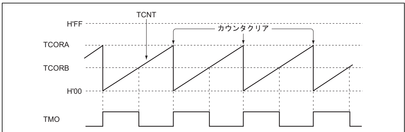
図 11.3 パルス出力例
