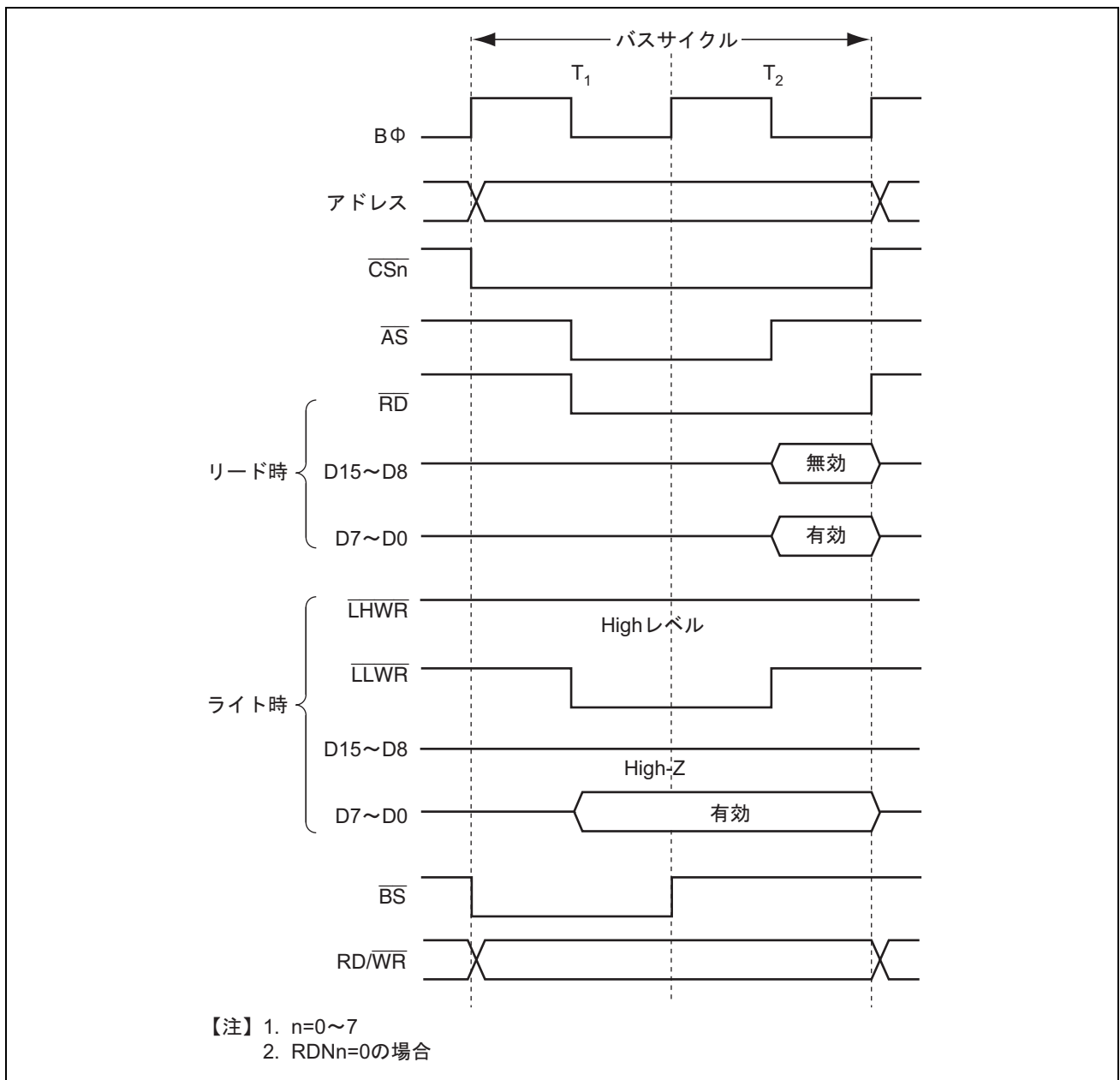
図 6.15 16 ビット 2 ステートアクセス空間のバスタイミング (奇数アドレスバイトアクセス)
