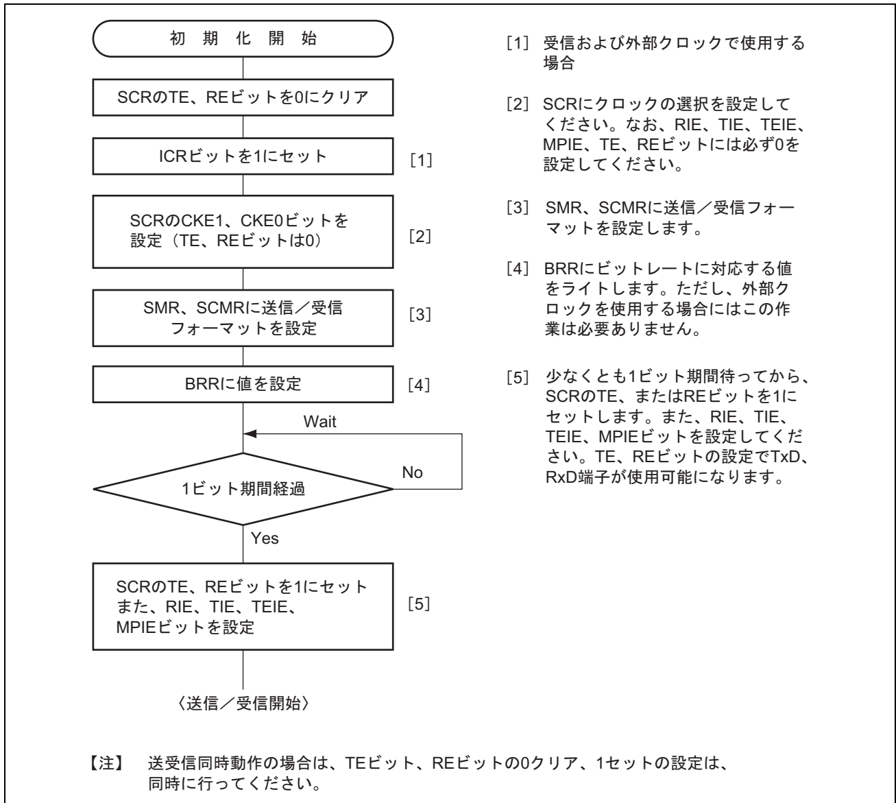
図 13.15 SCI の初期化フローチャートの例
