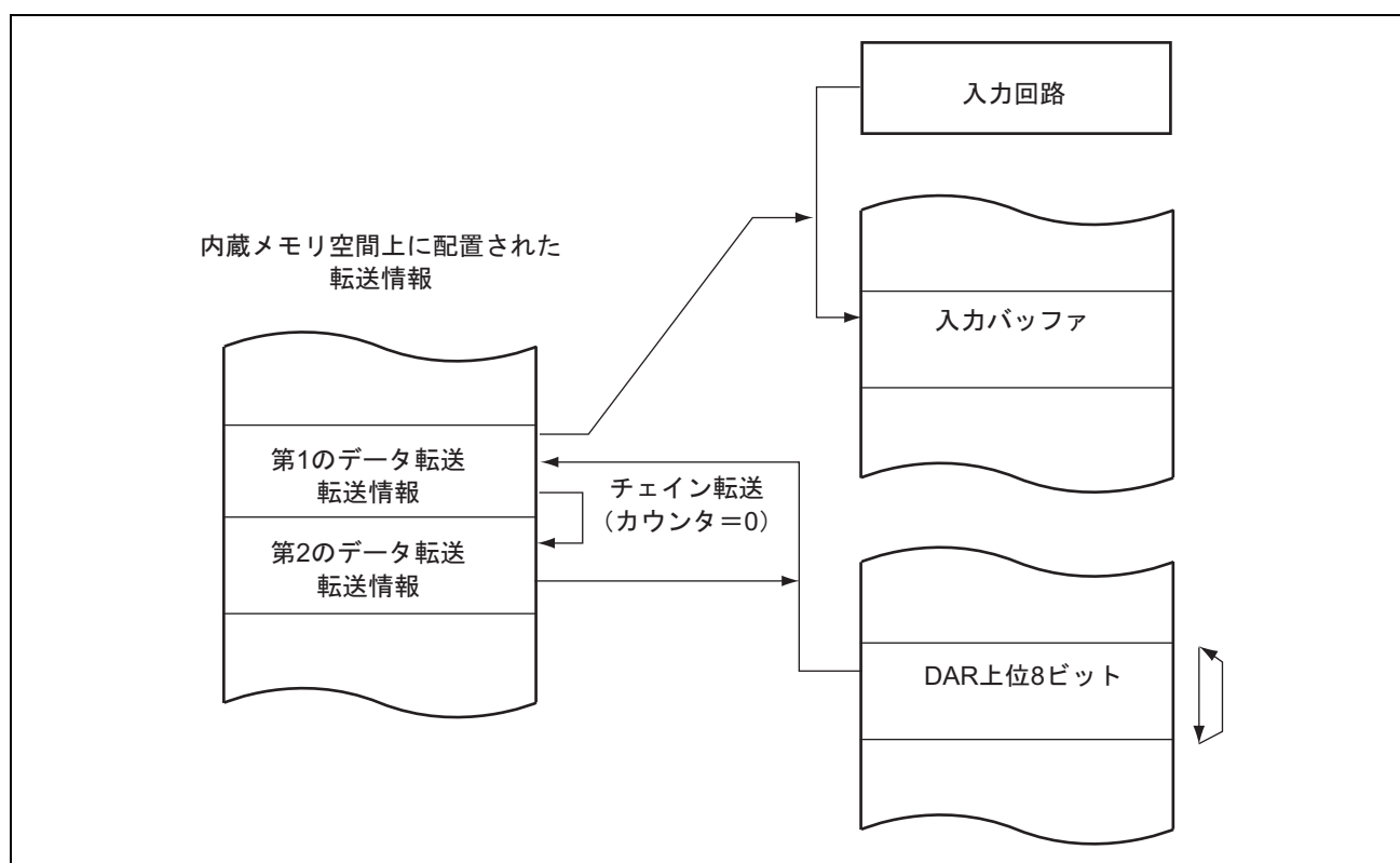
図 7.16 カウンタ=0 時のチェーン転送
