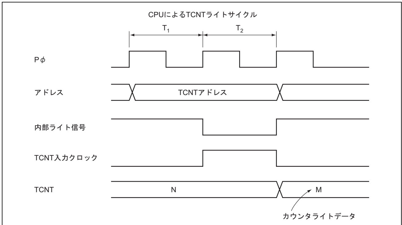
図 11.14 TCNT のライトとカウントアップの競合
