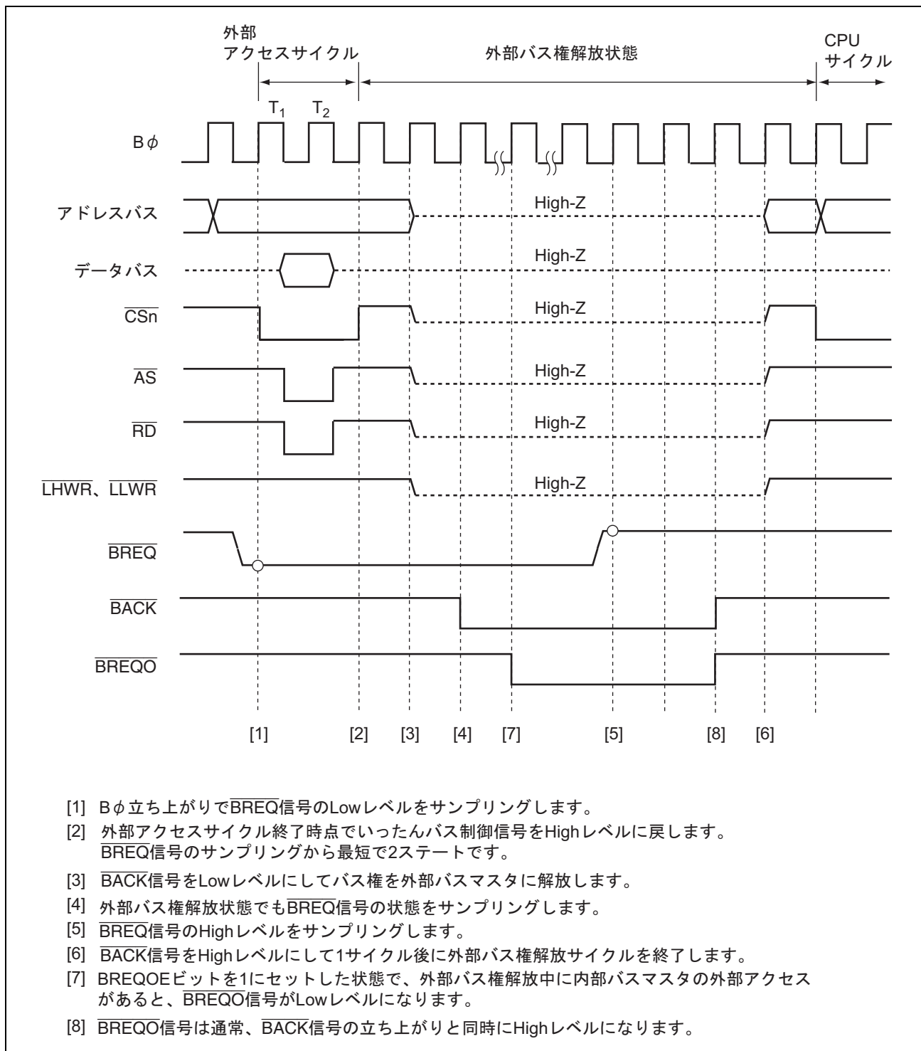
図 6.39 バス権解放状態遷移タイミング
