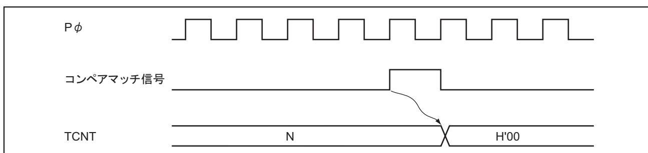
図 11.9 コンペアマッチによるカウンタクリアタイミング
