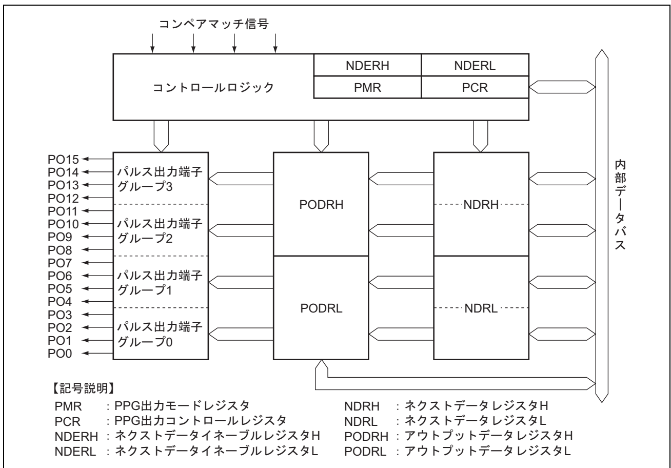
図 10.1 PPG のブロック図
