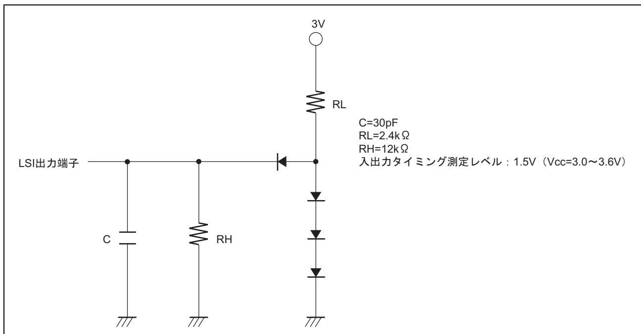
図 20.1 出力負荷回路
