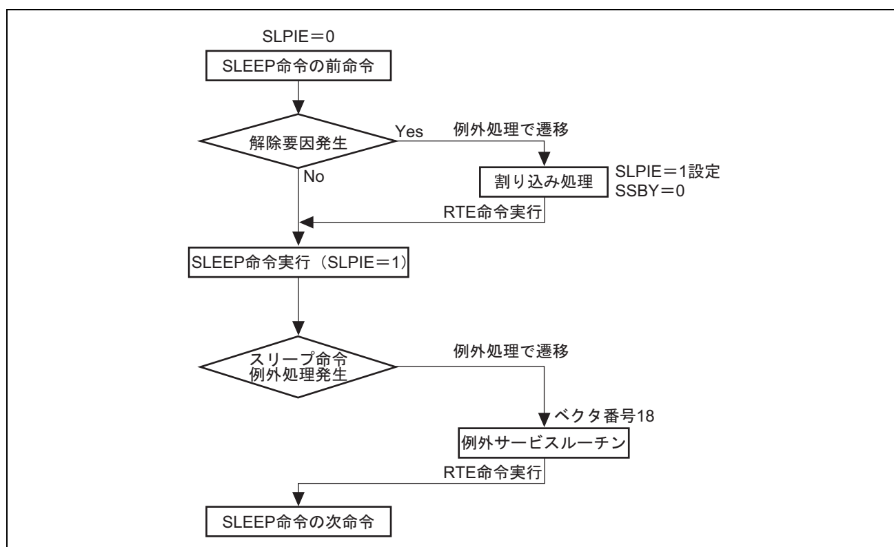
図 18.7 SLEEP 命令実行直前に解除要因割り込みが発生した場合（スリープ命令例外処理が発生する場合）
