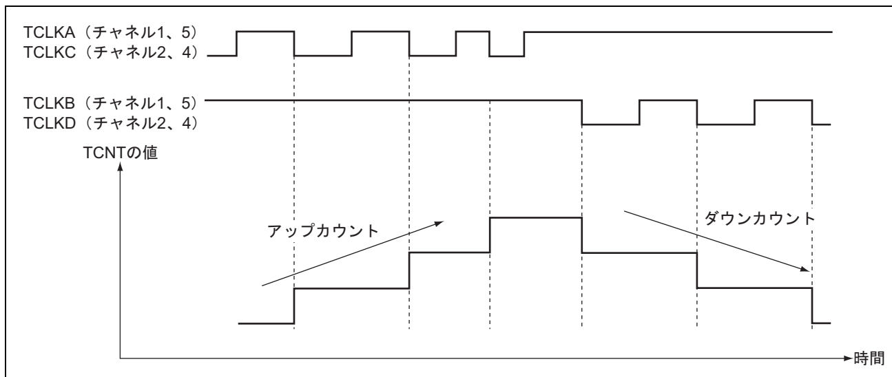
図 9.27 位相計数モード 3 の動作例
