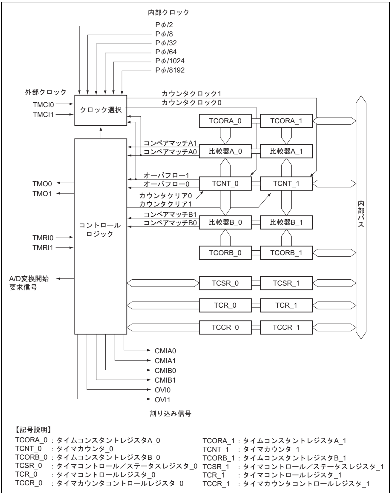
図 11.1 8ビットタイマ (ユニット0) のブロック図
