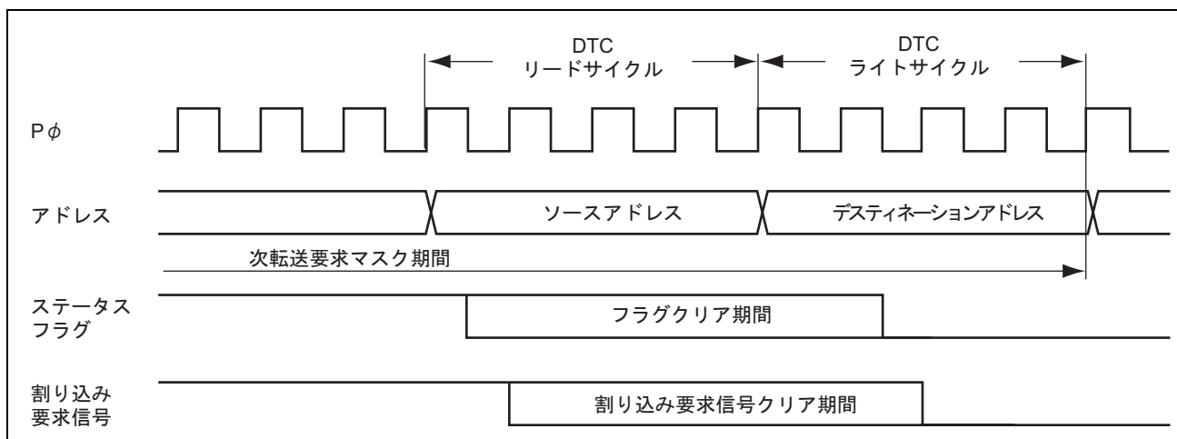
図 9.44 DTC の起動によるステータスフラグのクリアタイミング例 (2)
