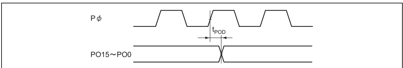
図 20.24 PPG 出力タイミング
