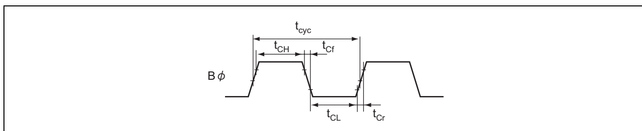
図 20.2 外部バスクロックタイミング
