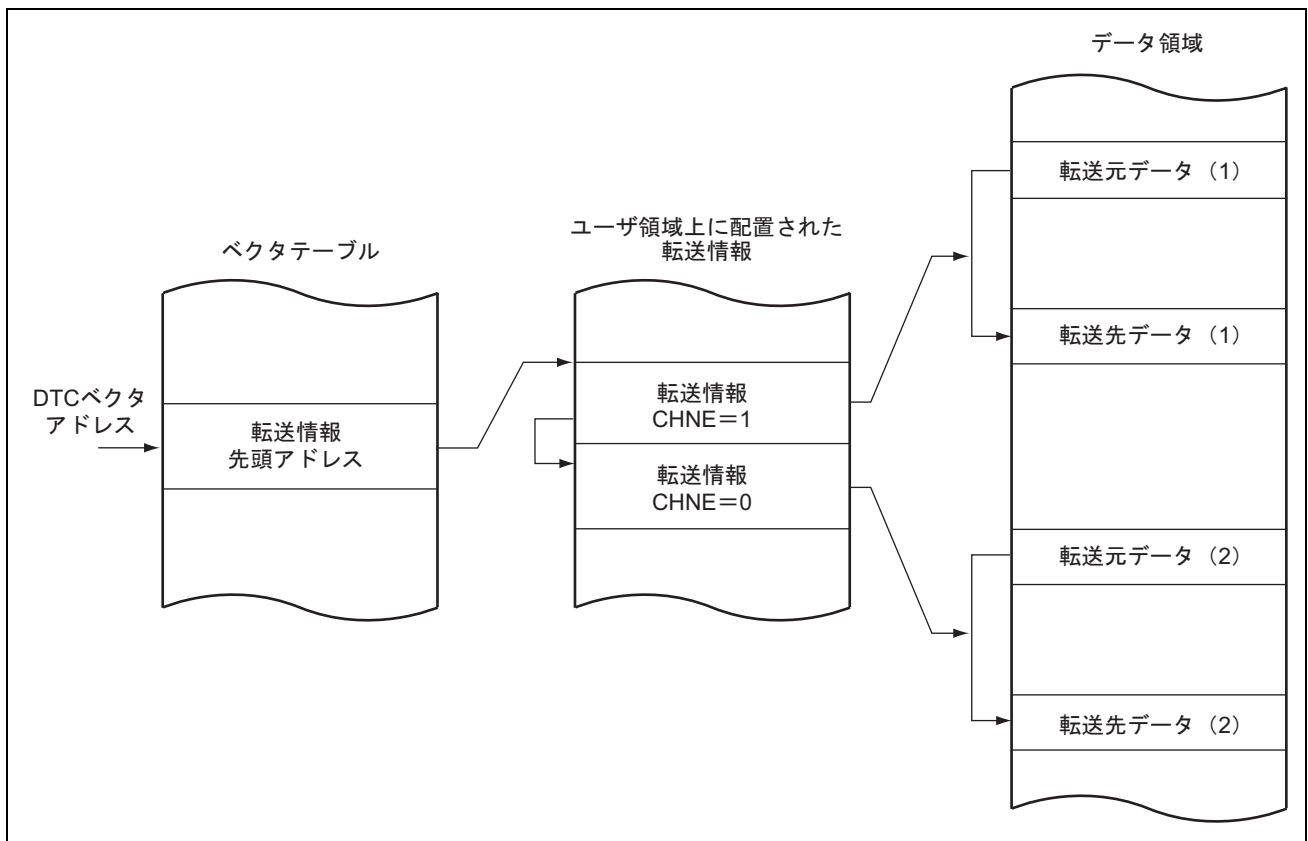
図 7.10 チェイン転送の動作
