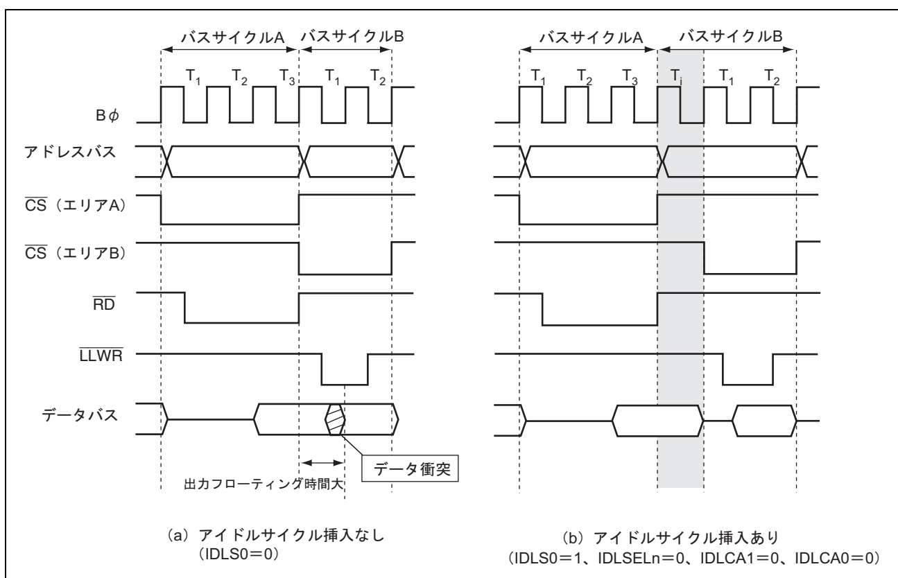
図 6.35 アイドルサイクル動作例 (リード後のライト)
