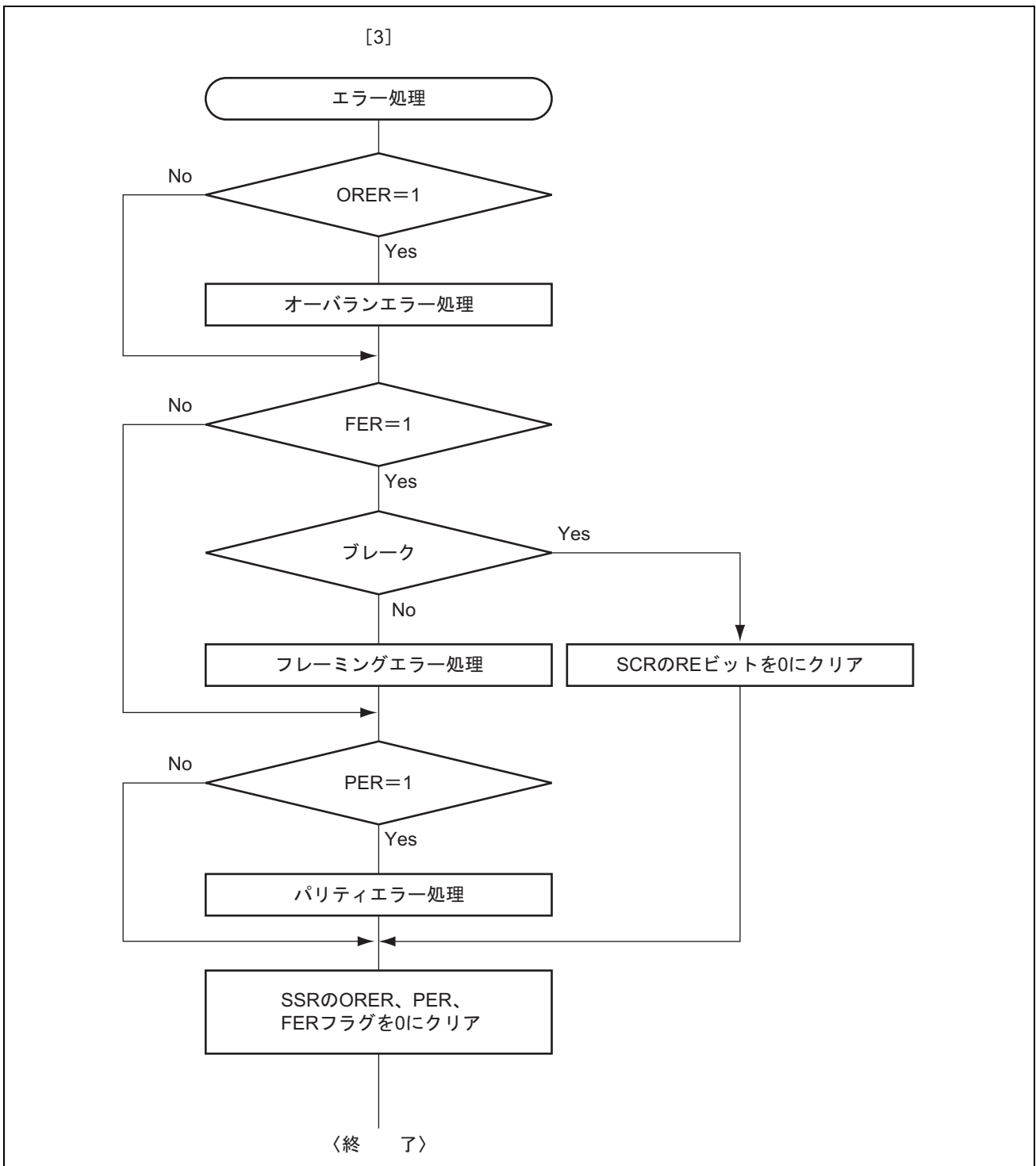
図 13.9 シリアル受信のフローチャートの例 (2)
