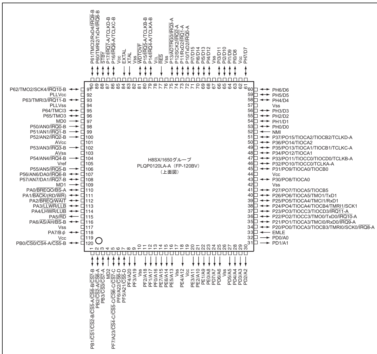
図 1.3 ピン配置図
