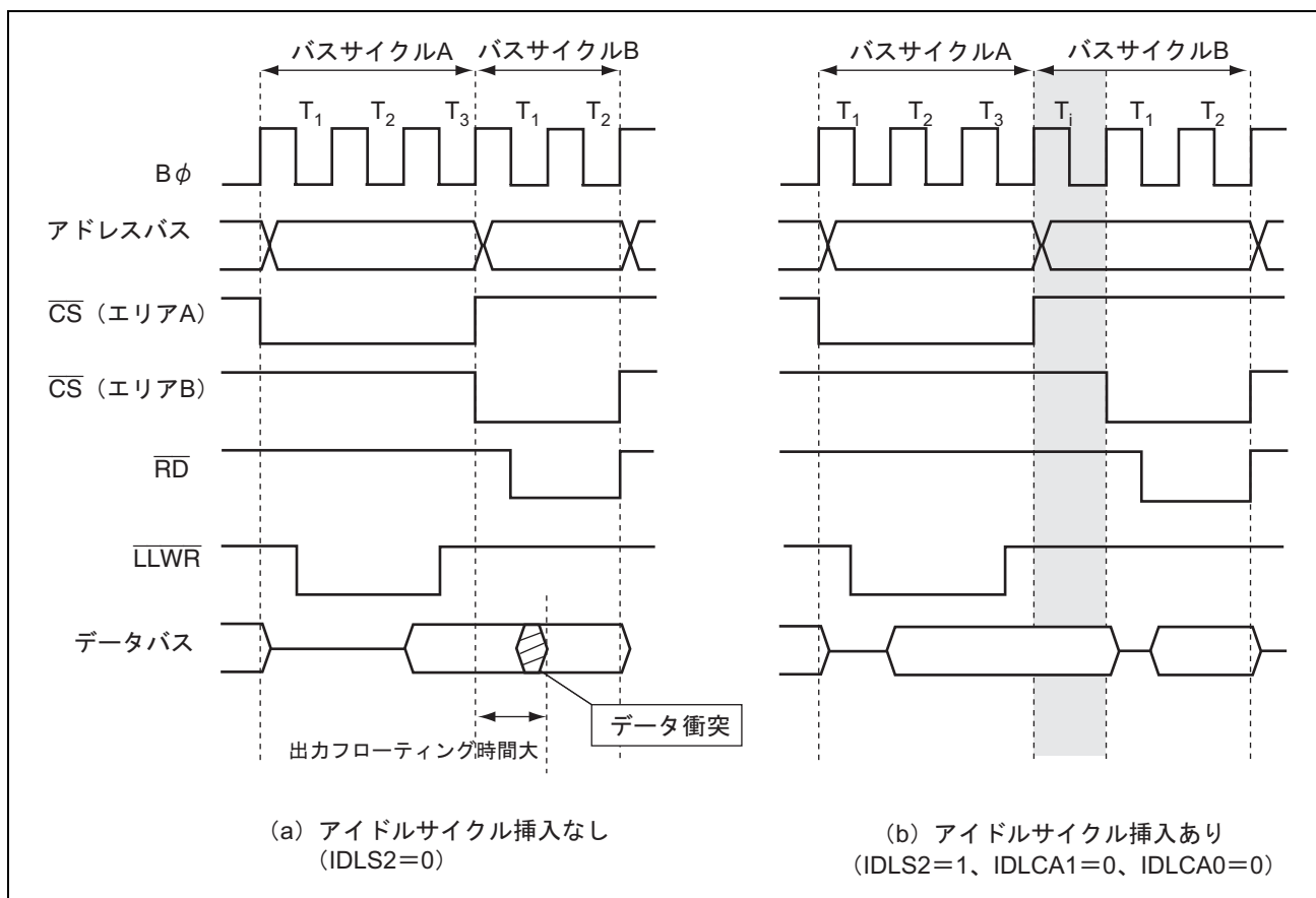
図 6.36 アイドルサイクル動作例 (ライト後のリード)
