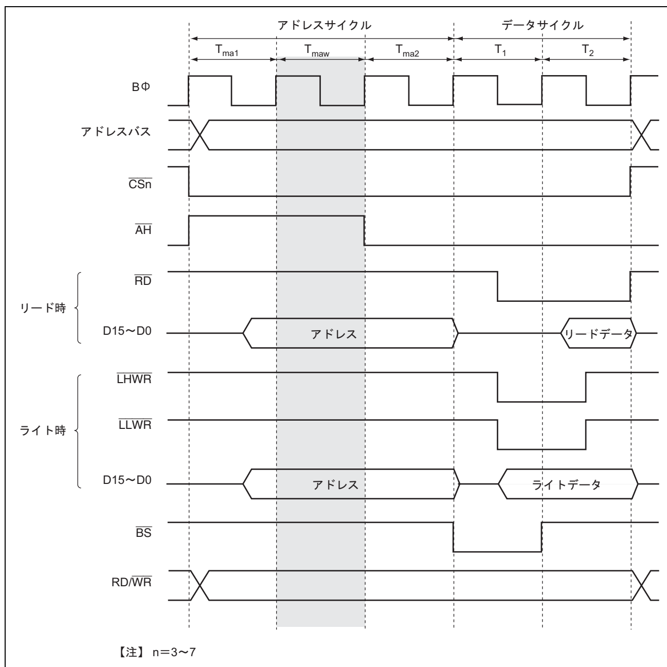
図 6.30 アドレスサイクル 3 サイクルのアクセスタイミング例 (ADDEX=1)
