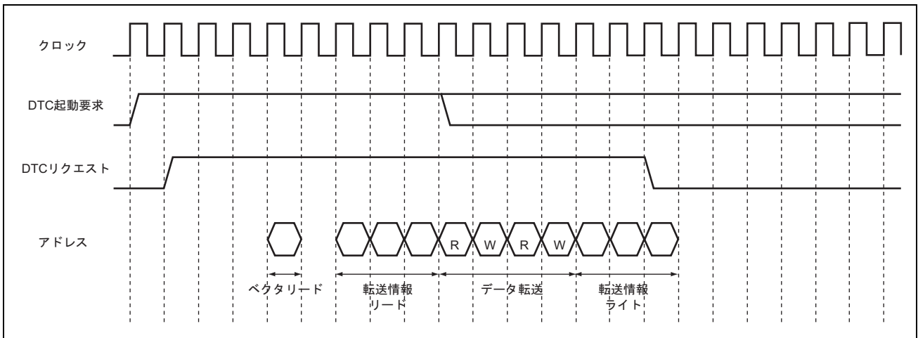
図 7.12 DTC の動作タイミング例 (ショートアドレスモード、ブロック転送モード、ブロックサイズ=2)
