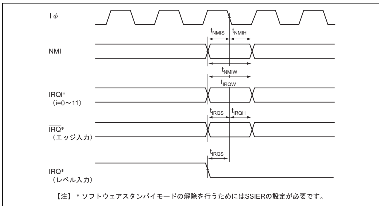
図 20.7 割り込み入力タイミング
