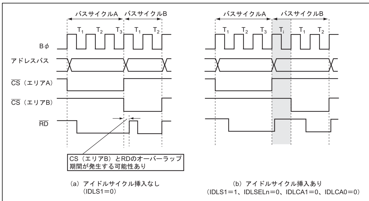
図 6.38 チップセレクト ( \overline{CS} ) とリード ( \overline{RD} ) の関係
