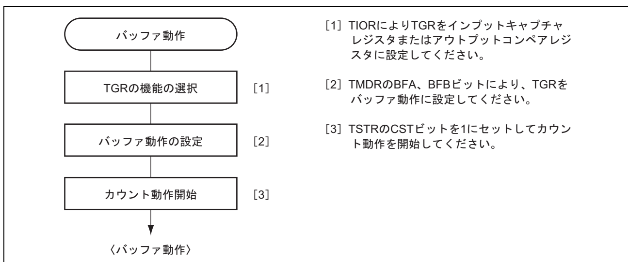
図 9.14 バッファ動作の設定手順例
