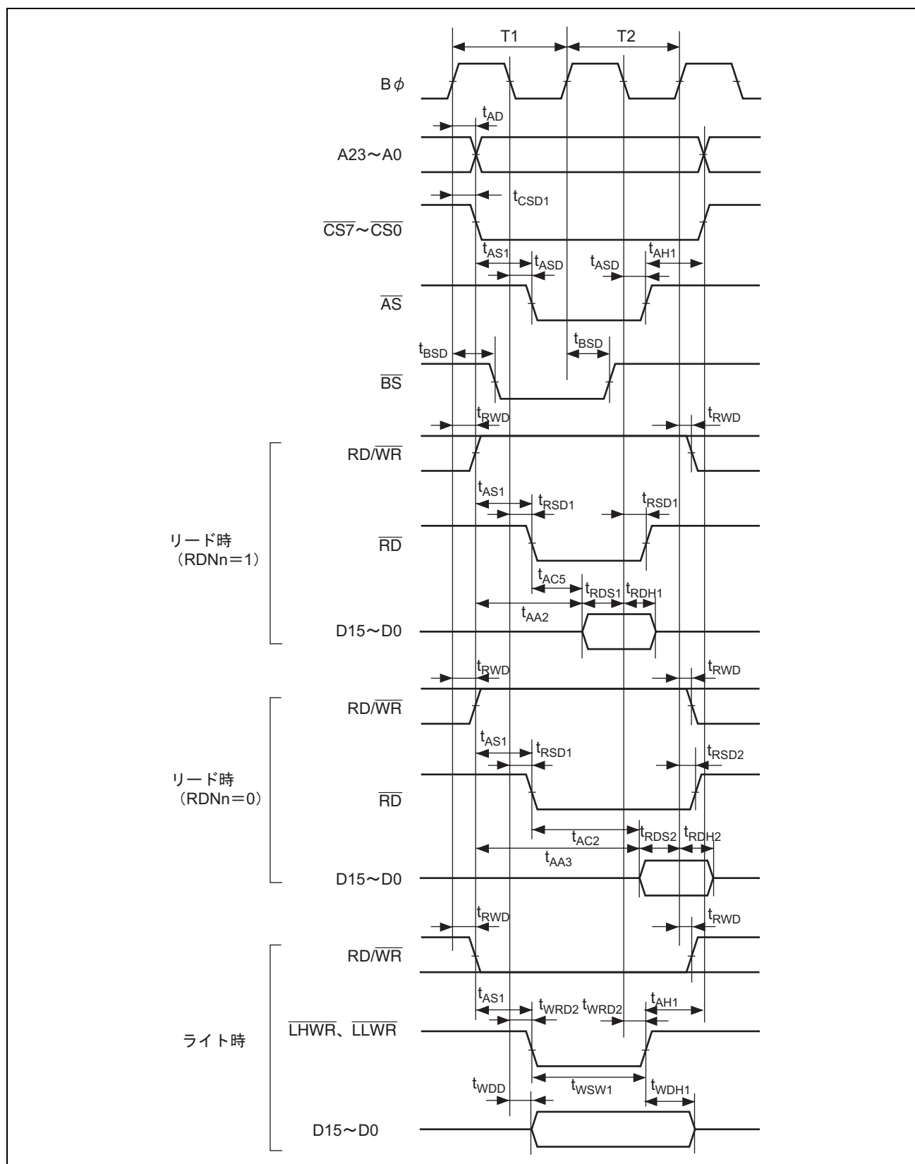
図 20.8 基本バスタイミング/2 ステートアクセス
