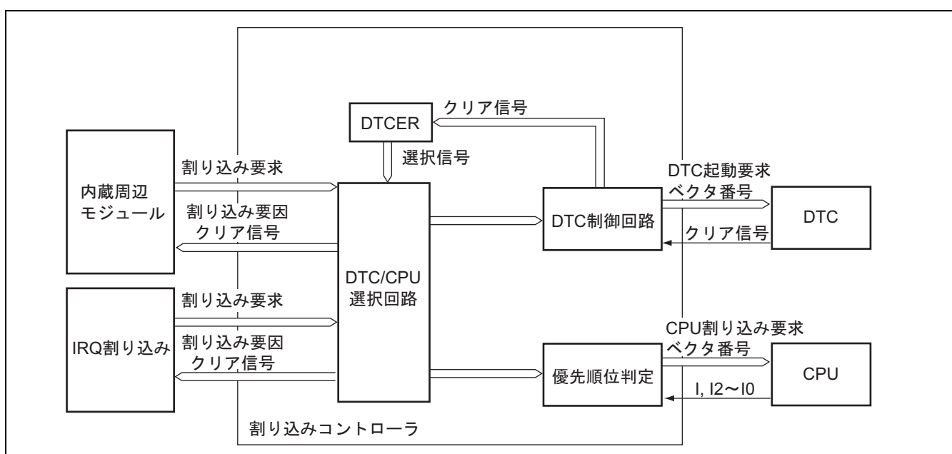
図 5.6 DTC と割り込みコントローラ
