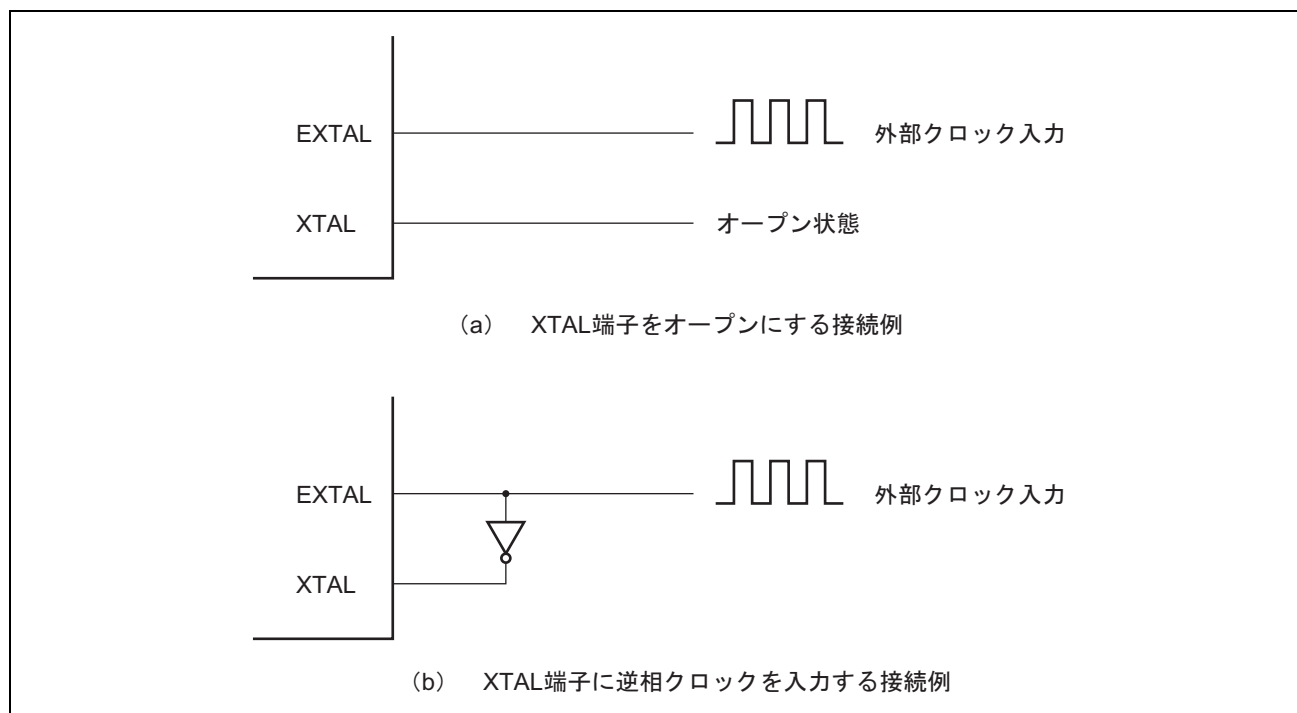
図 17.4 外部クロックの接続例
