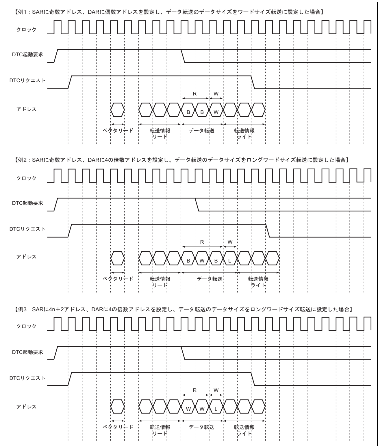
図 7.5 バスサイクルが分割される例
