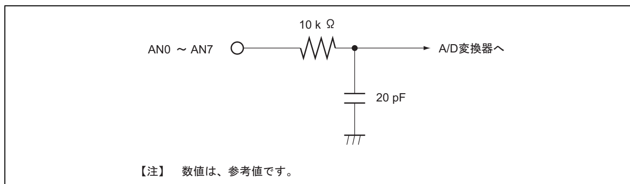
図 14.10 アナログ入力端子等価回路
