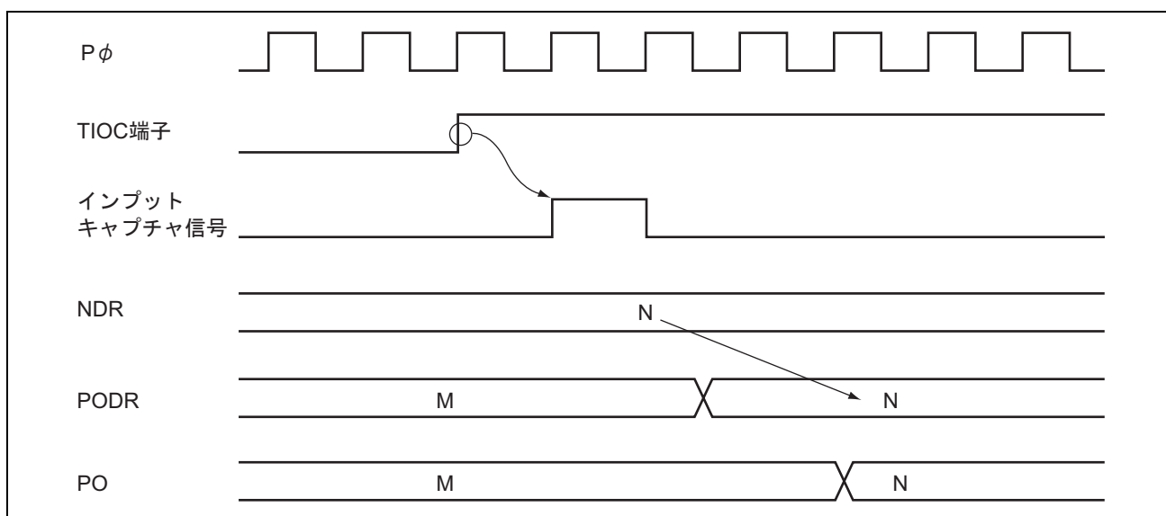
図 10.11 インพุットキャプチャによるパルス出力例
