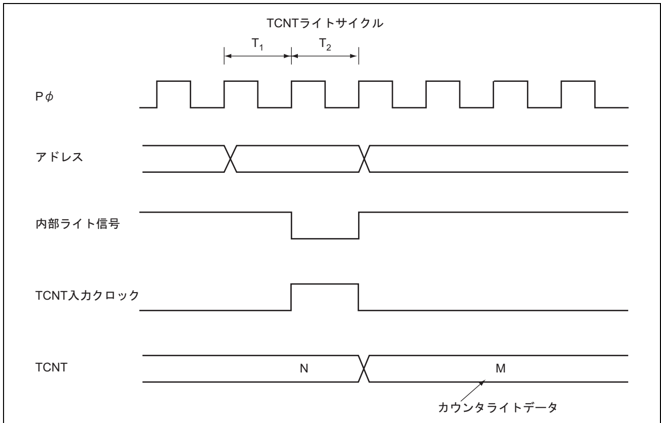
図 12.5 TCNT のライトとカウントアップの競合
