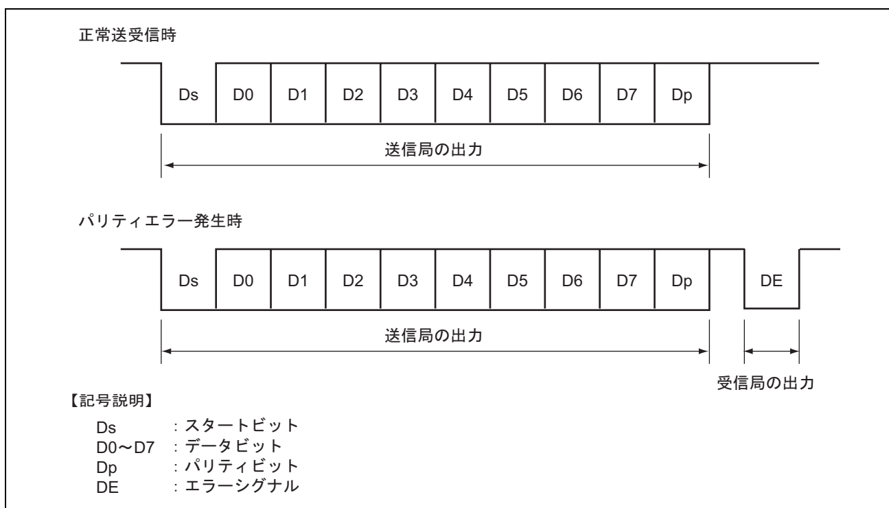
図 13.22 通常のスマートカードインタフェースのデータフォーマット
