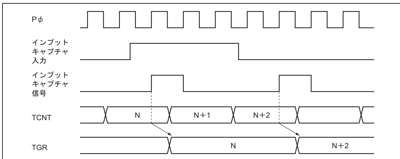
図 9.33 インพุットキャプチャ入力信号タイミング
