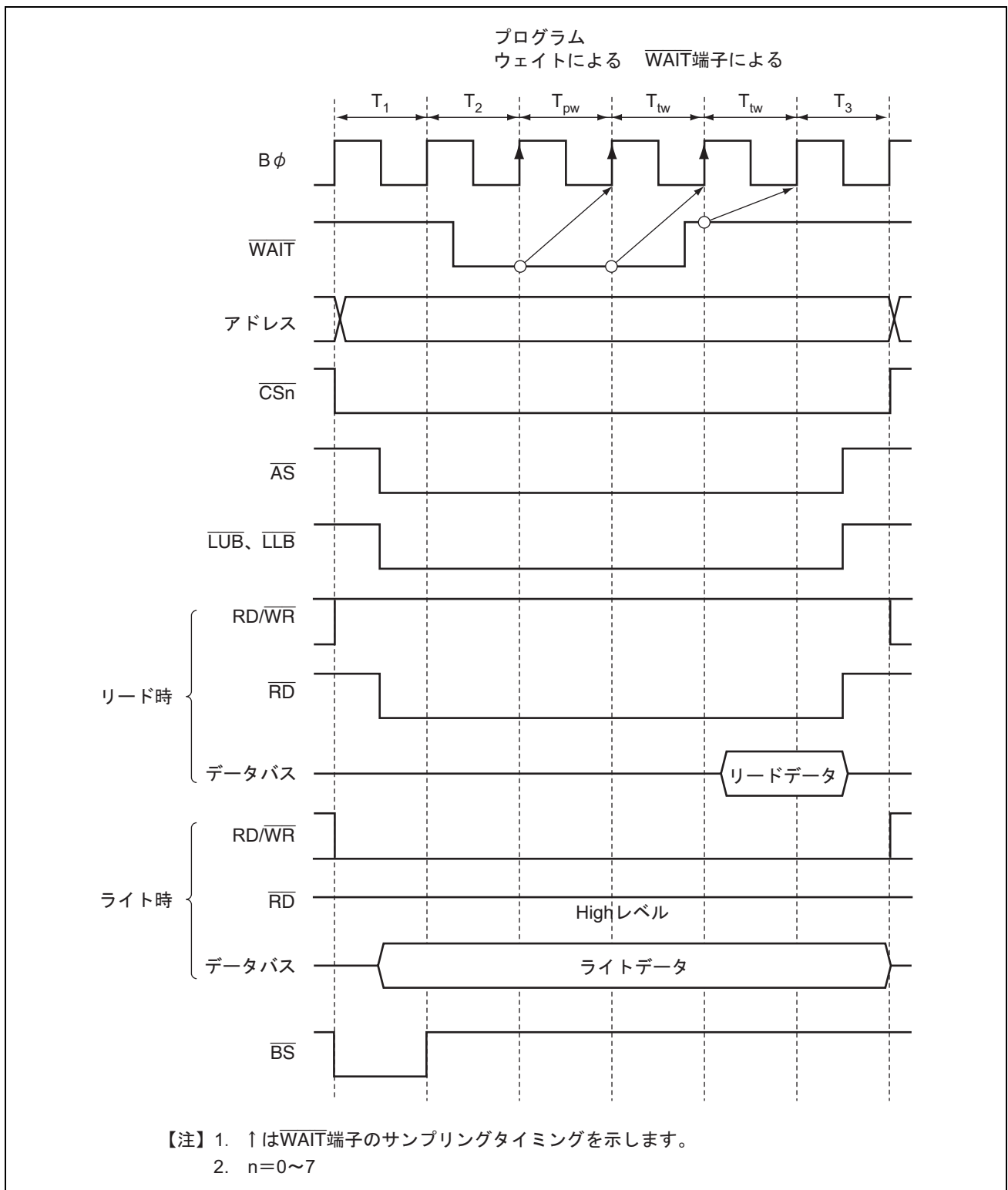
図 6.25 ウェイトステート挿入のタイミング例
