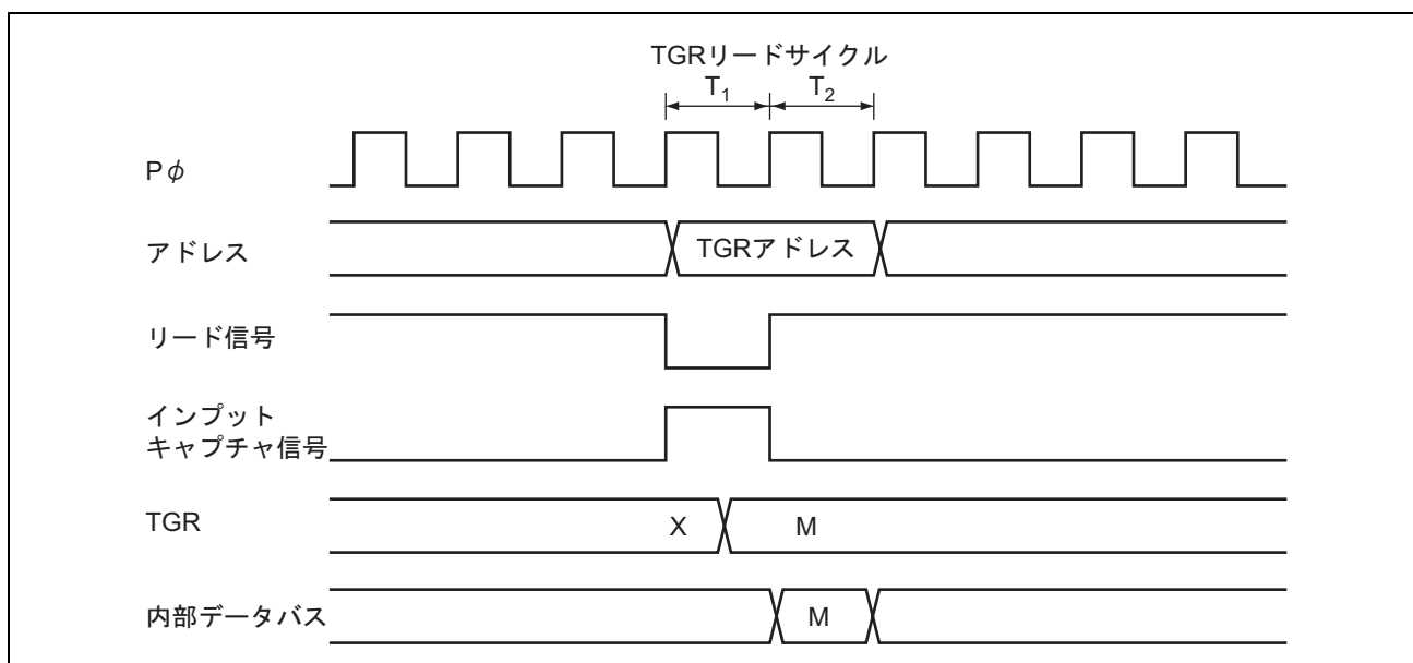
図 9.50 TGRのリードとインプットキャプチャの競合
