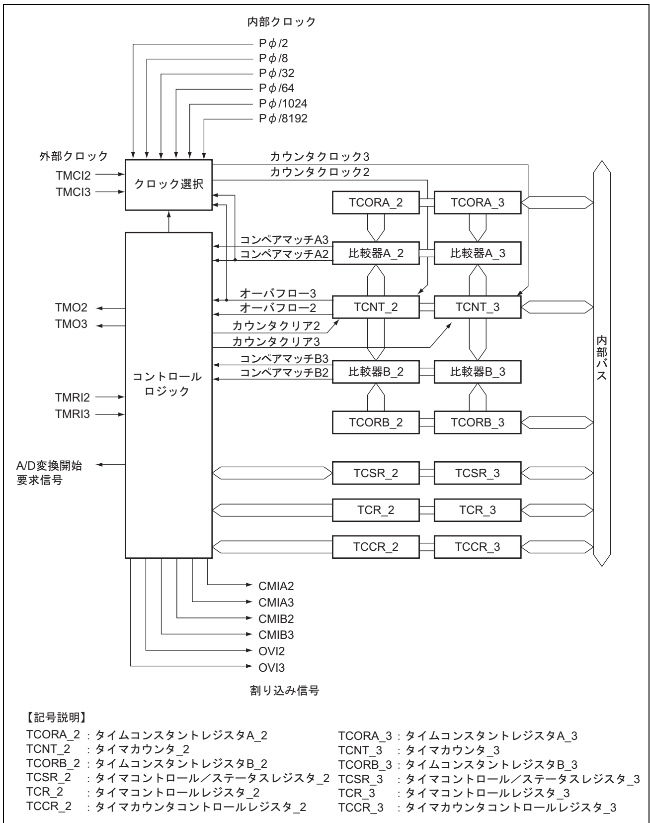
図 11.2 8ビットタイマ (ユニット1) のブロック図
