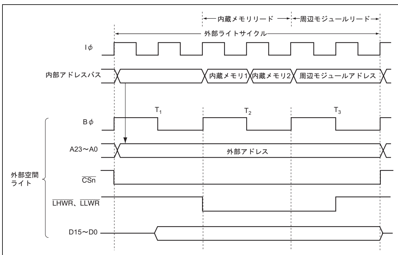
図 6.40 外部ライトバッファ機能使用時のタイミング例
