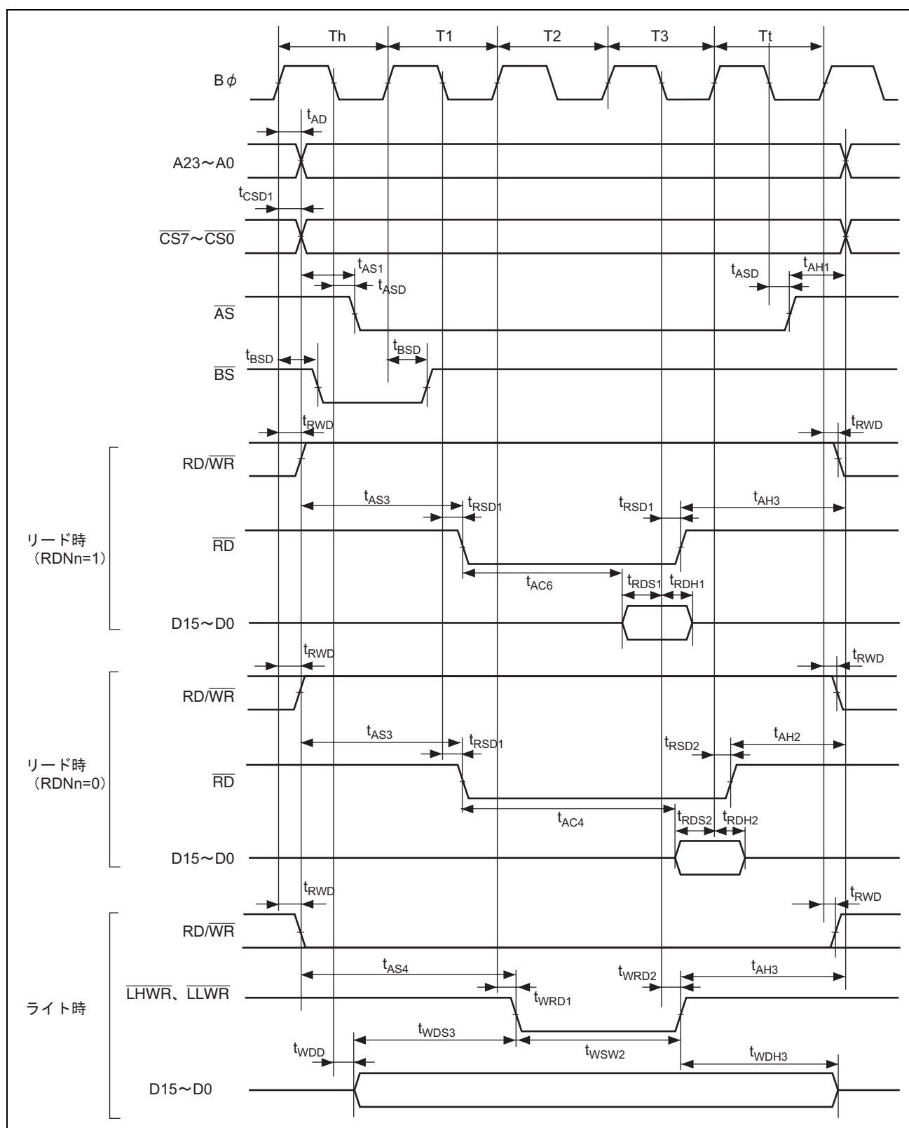
図 20.12 基本バスタイミング/3 ステートアクセス ( \overline{CS} アサート期間延長)
