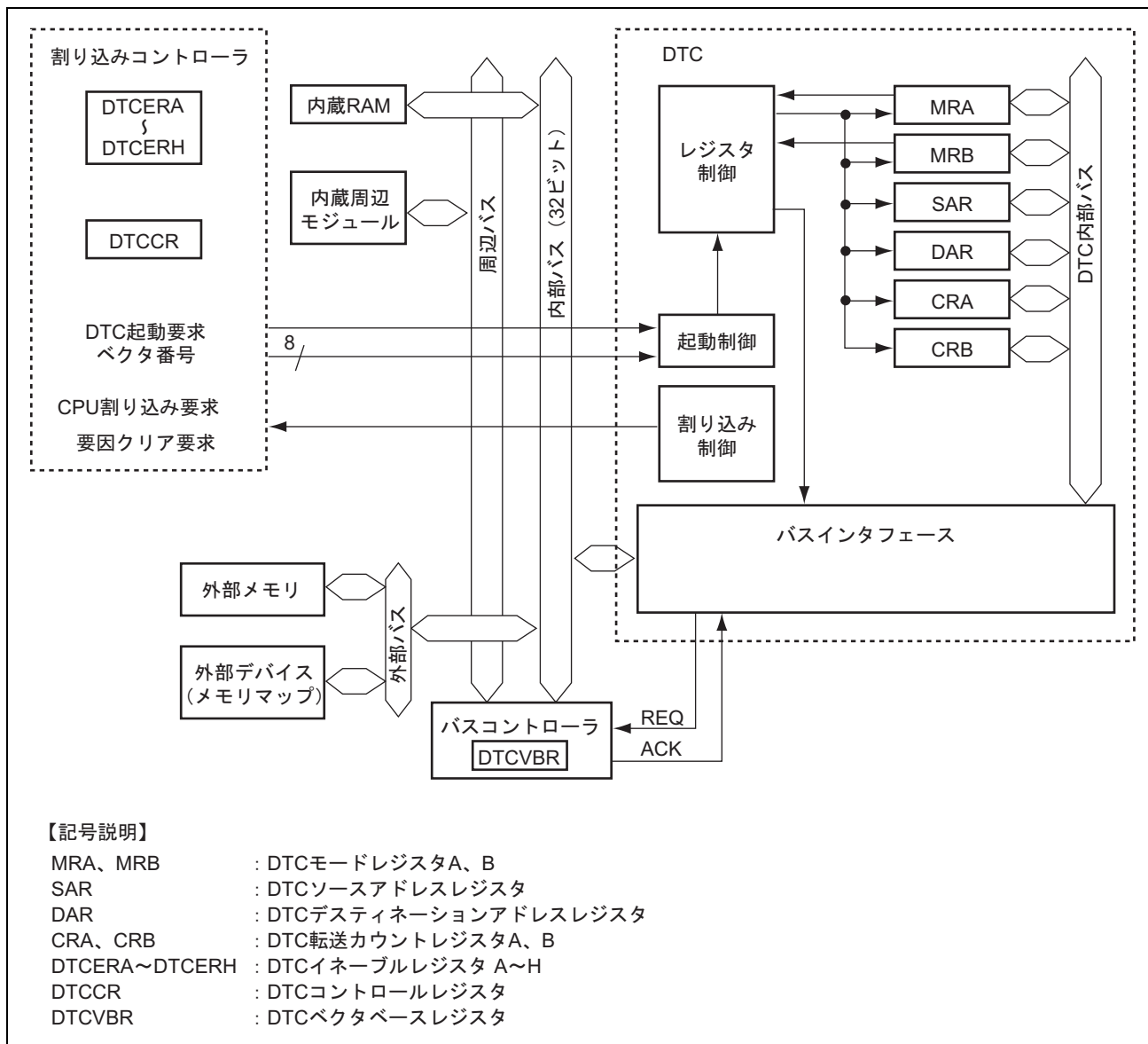
図 7.1 DTC のブロック図
