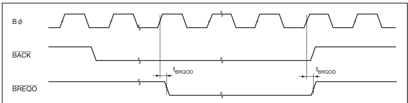
図 20.20 外部バス権要求出力タイミング
