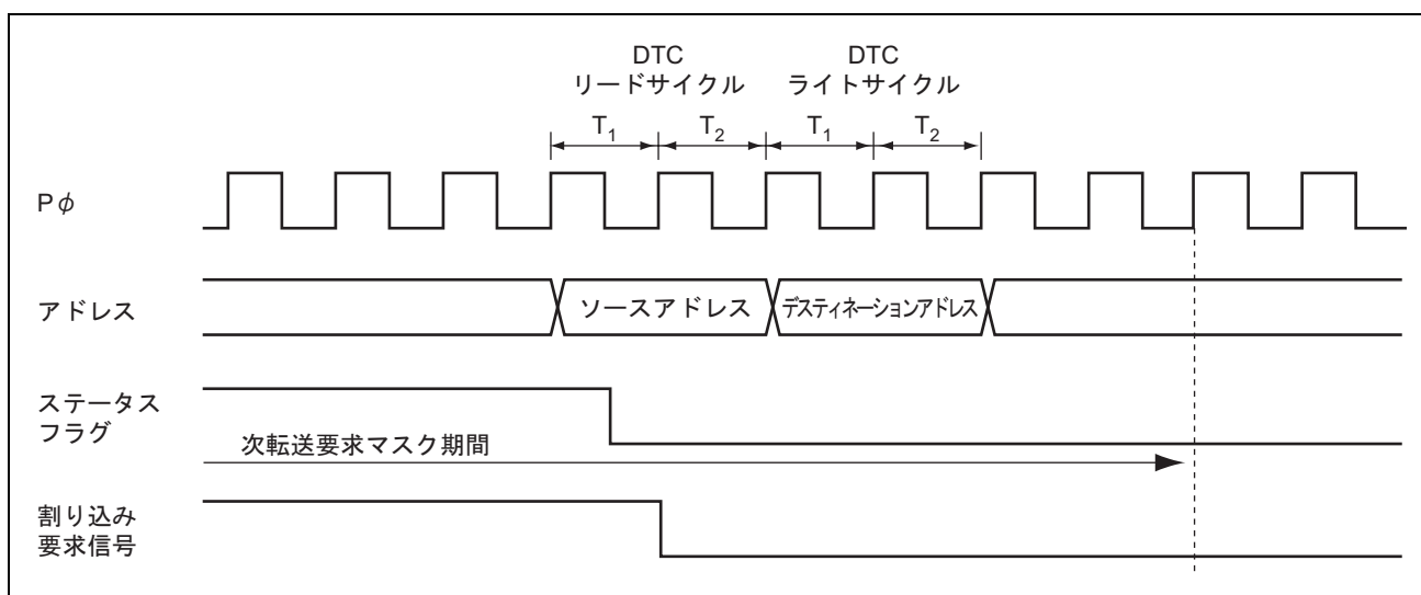
図 9.43 DTCの起動によるステータスフラグのクリアタイミング例 (1)
