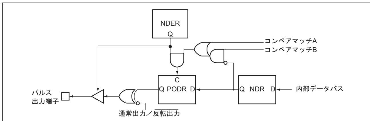
図 10.6 パルス出力ノンオーバーラップ動作
