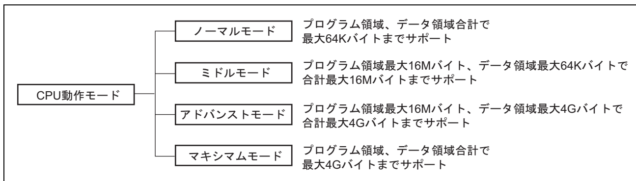
図 2.1 CPU 動作モード
