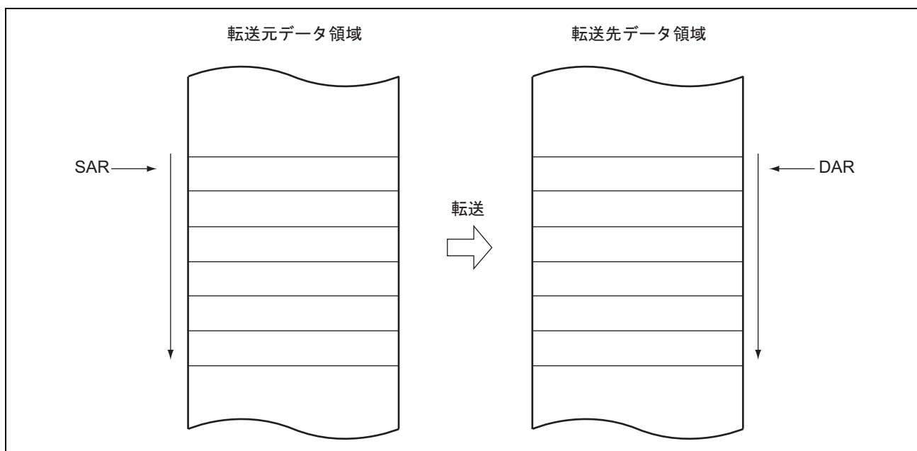
図 7.7 ノーマル転送モードのメモリマップ
