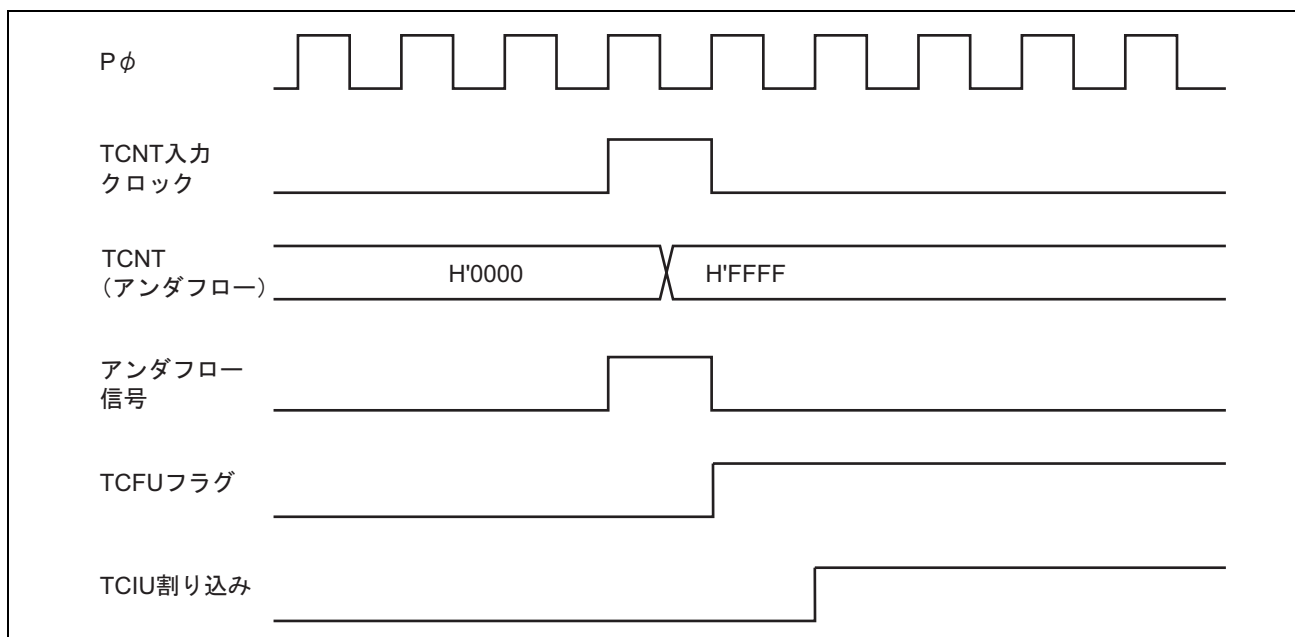
図 9.41 TCIU 割り込みのセットタイミング
