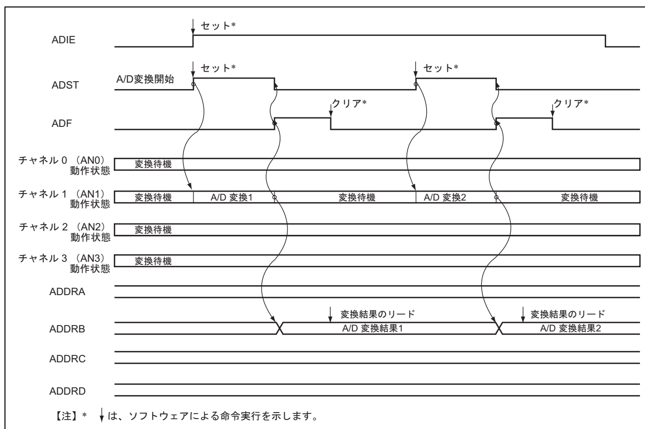
図 14.2 A/D 変換器の動作例（シングルモード、チャンネル 1 選択時）
