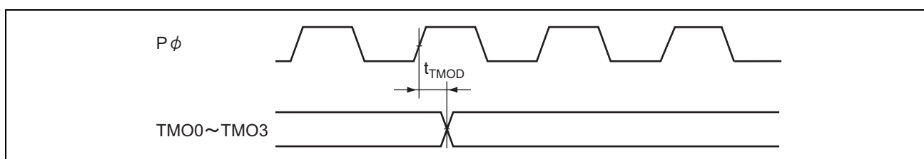
図 20.25 8ビットタイマ出力タイミング
