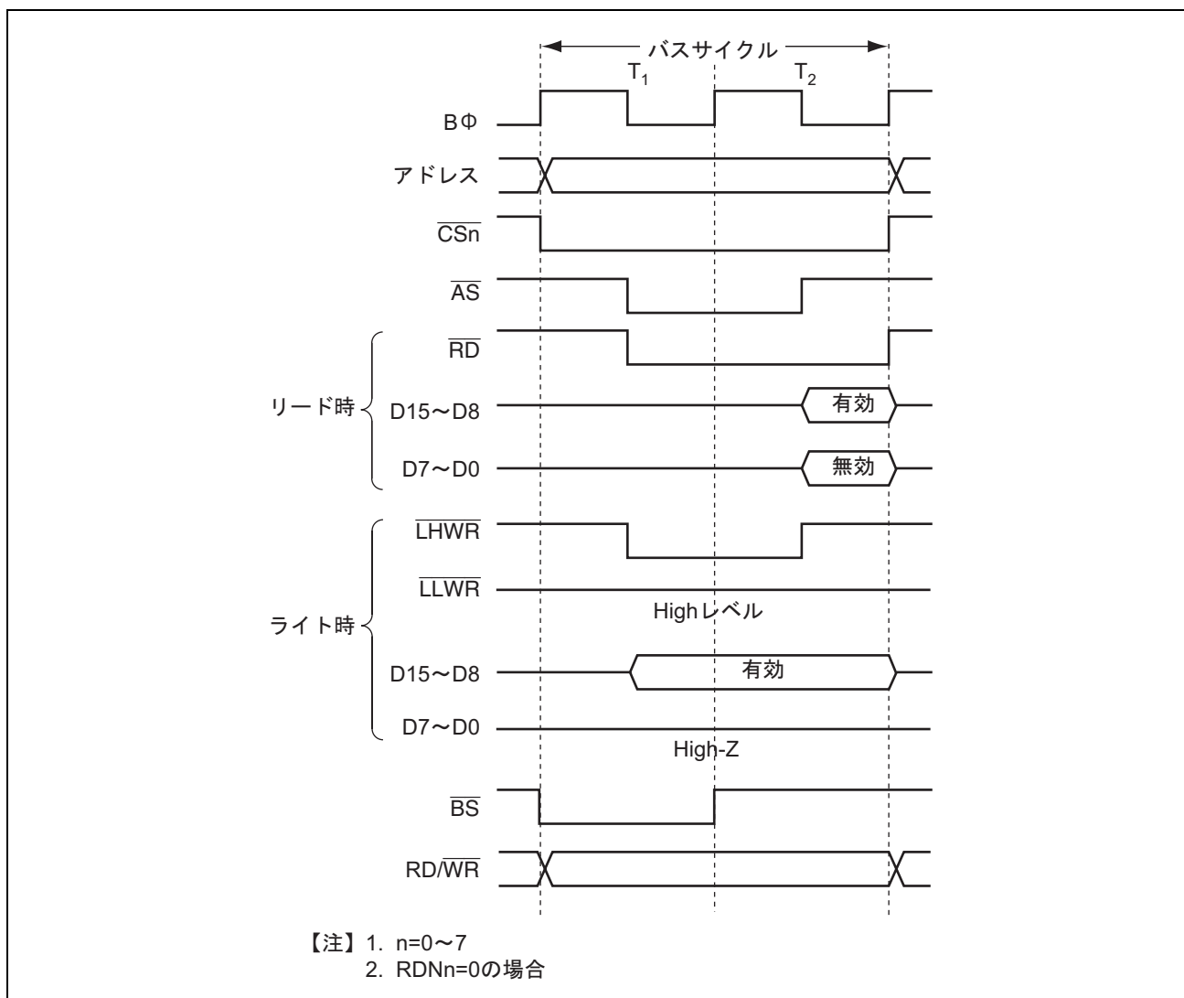
図 6.14 16 ビット 2 ステートアクセス空間のバスタイミング (偶数アドレスバイトアクセス)
