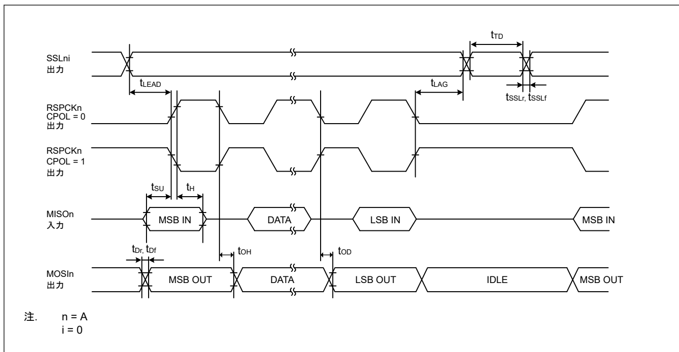
図 39.29 SPI タイミング (マスタ、CPHA = 0) (ビットレート : PCLKA を 2 分周以外に設定)
