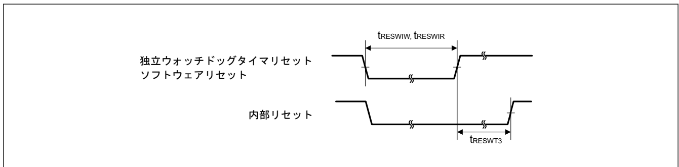
図 39.9 リセット入カタイミング (2)
