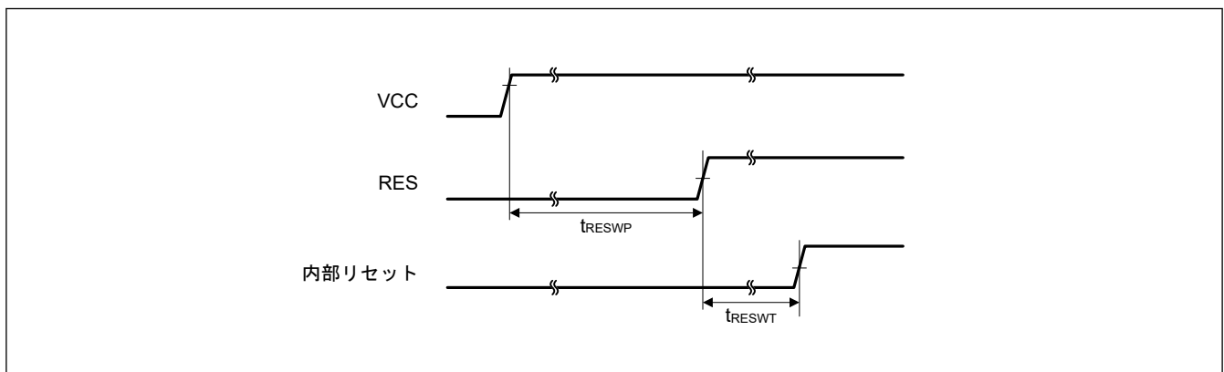
図 39.7 電源投入時リセット入カタイミング
