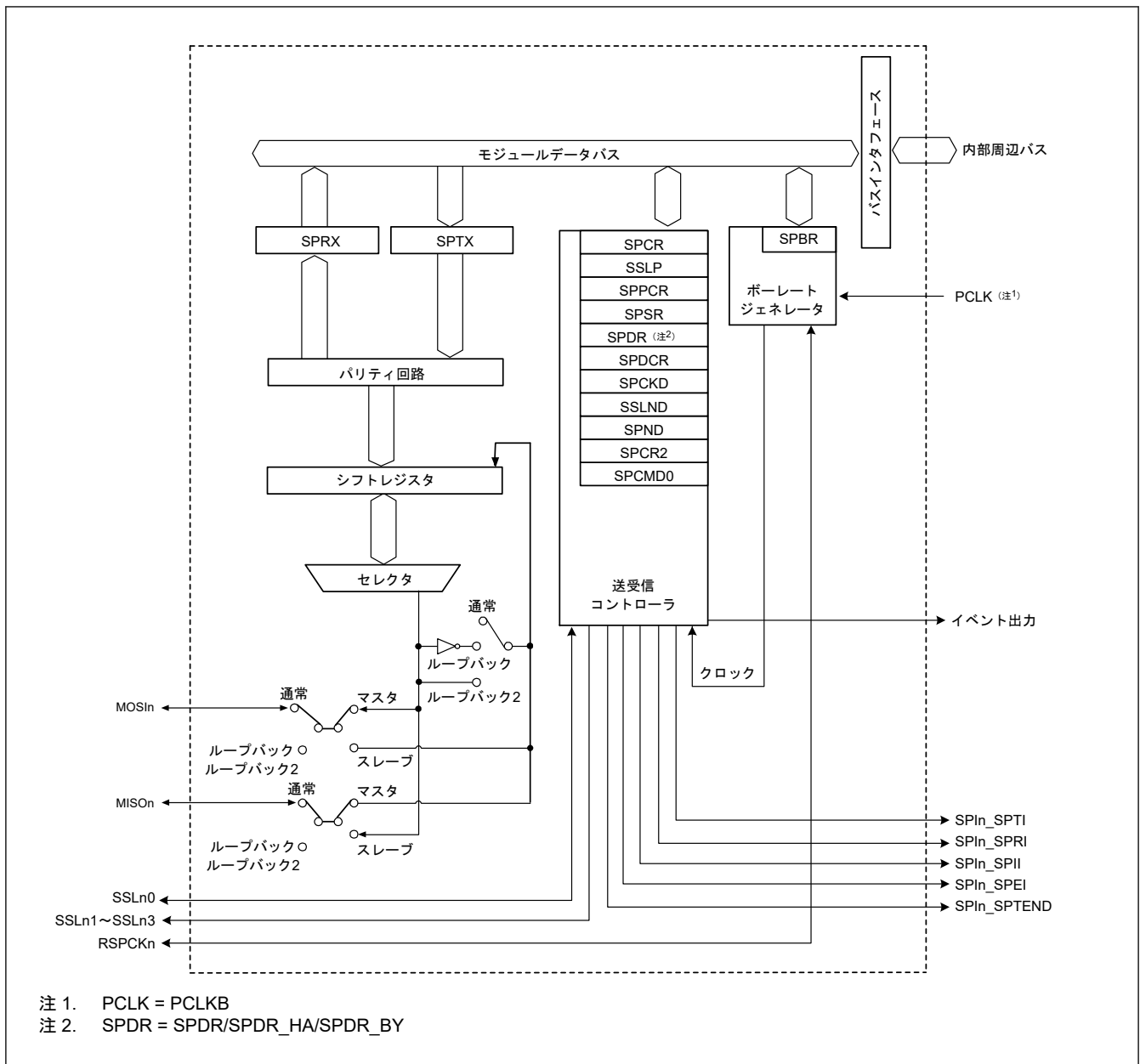
図 27.1 SPI のブロック図
