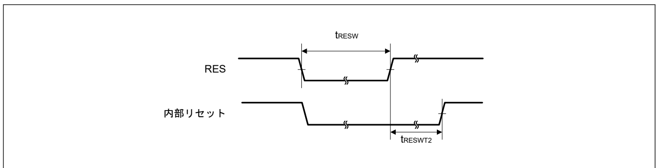
図 39.8 リセット入カタイミング (1)
