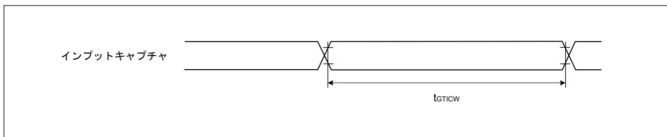
図 39.16 GPT 入力キャプチャタイミング
