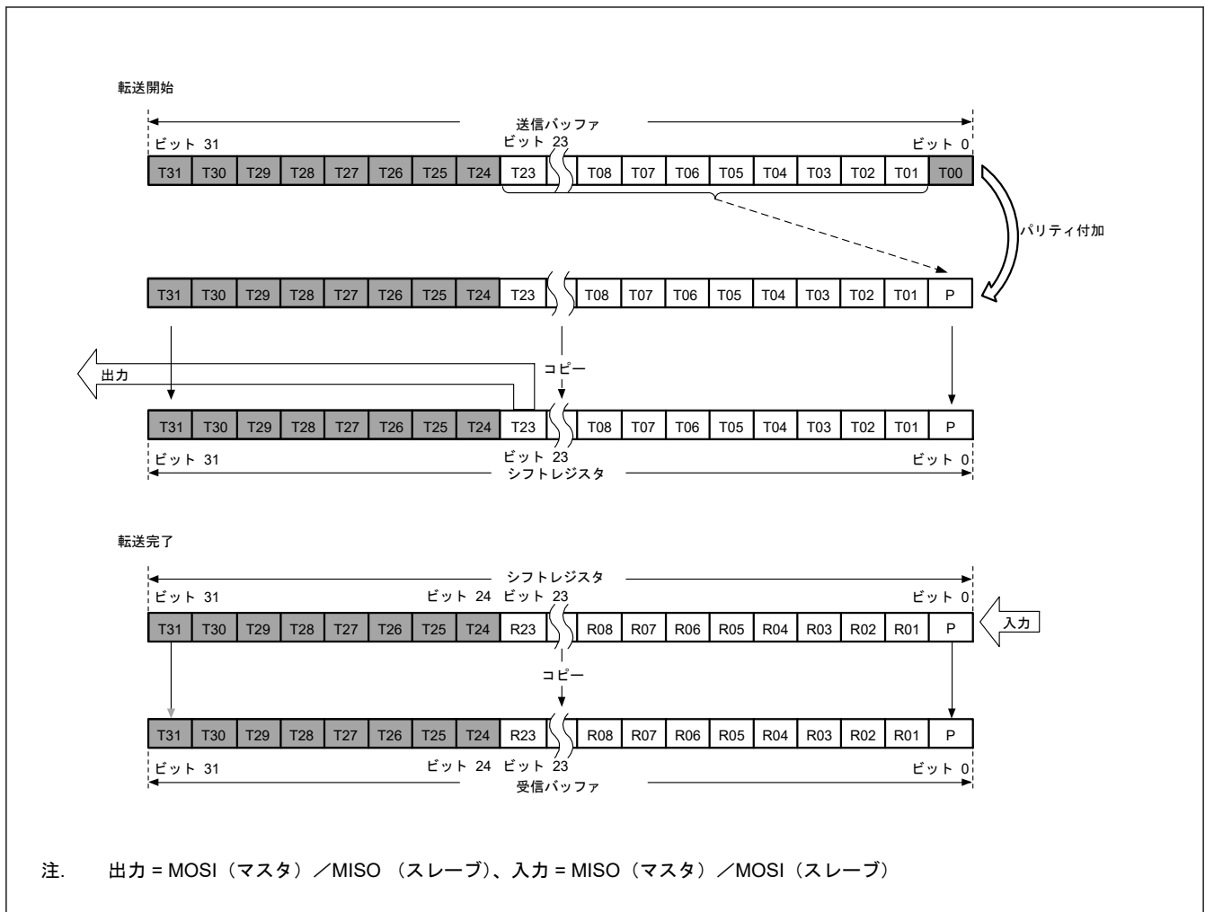
図 27.19 MSB ファースト転送 (24 ビットデータ/パリティ機能有効)
