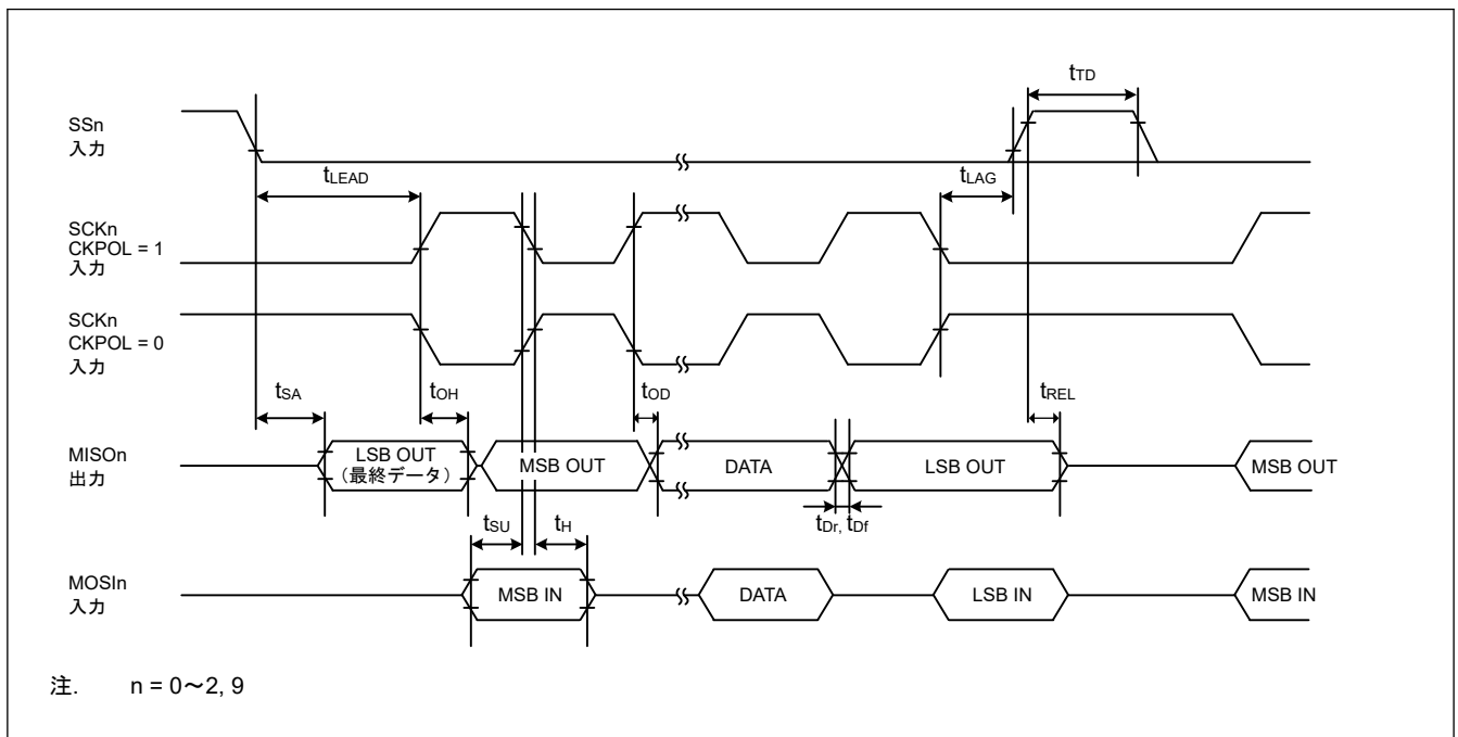
図 39.26 SCI 簡易 SPI モードタイミング (スレーブ、CKPH = 0)
