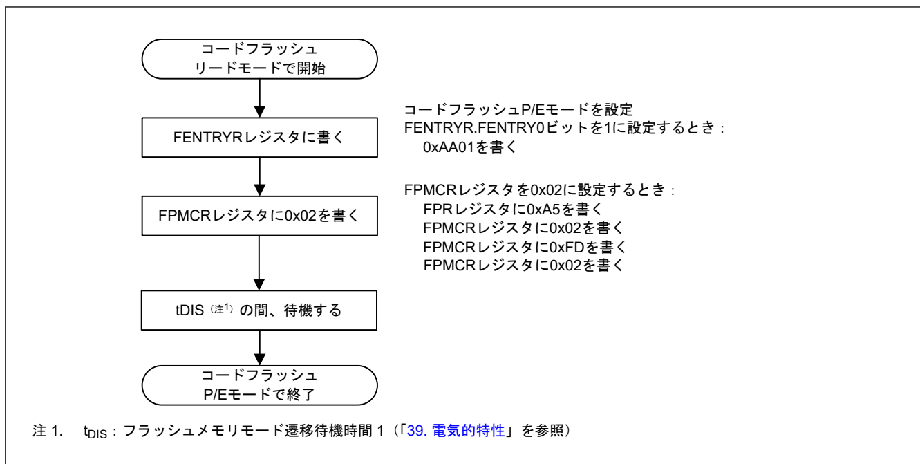
図 35.15 読み出しモードからコードフラッシュ P/E モードへの変更手順
