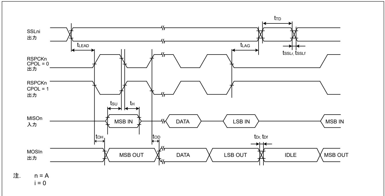
図 39.31 SPI タイミング (マスタ、CPHA = 1) (ビットレート : PCLKA を 2 分周以外に設定)
