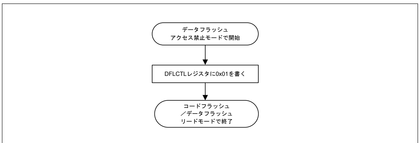
図 35.14 データフラッシュアクセス禁止モードから読み出しモードへのモード遷移
