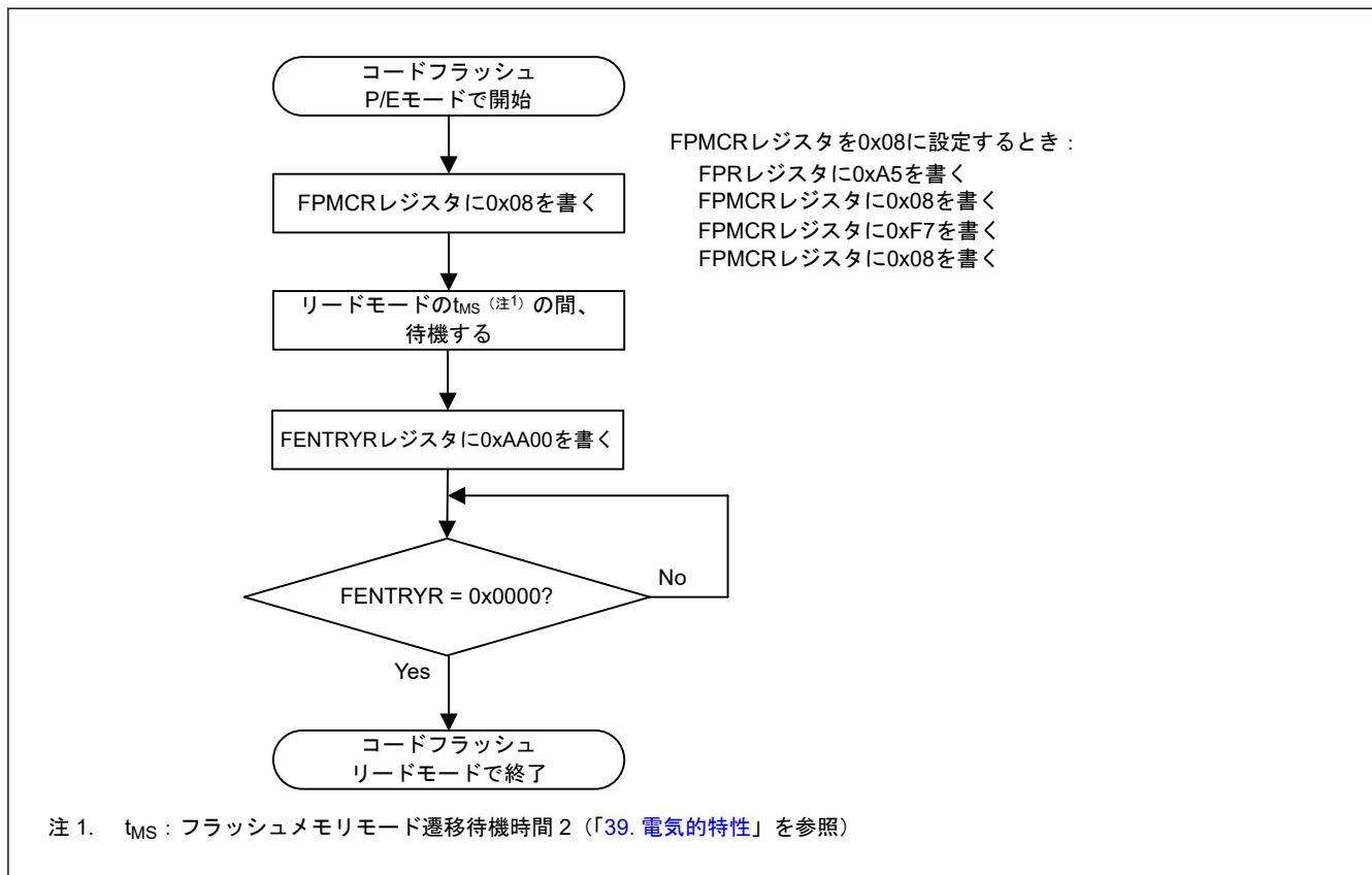
図 35.17 コードフラッシュ P/E モードから読み出しモードへの変更手順
