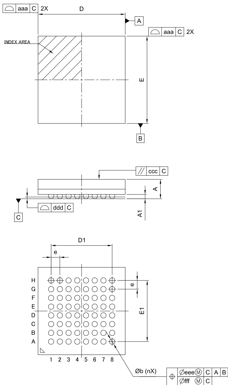
図 2.11 VFBGA 64 ピン
