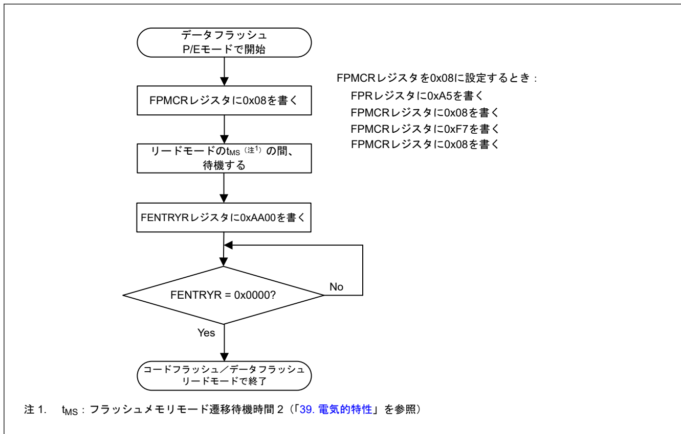
図 35.18 データフラッシュ P/E モードから読み出しモードへの変更手順
