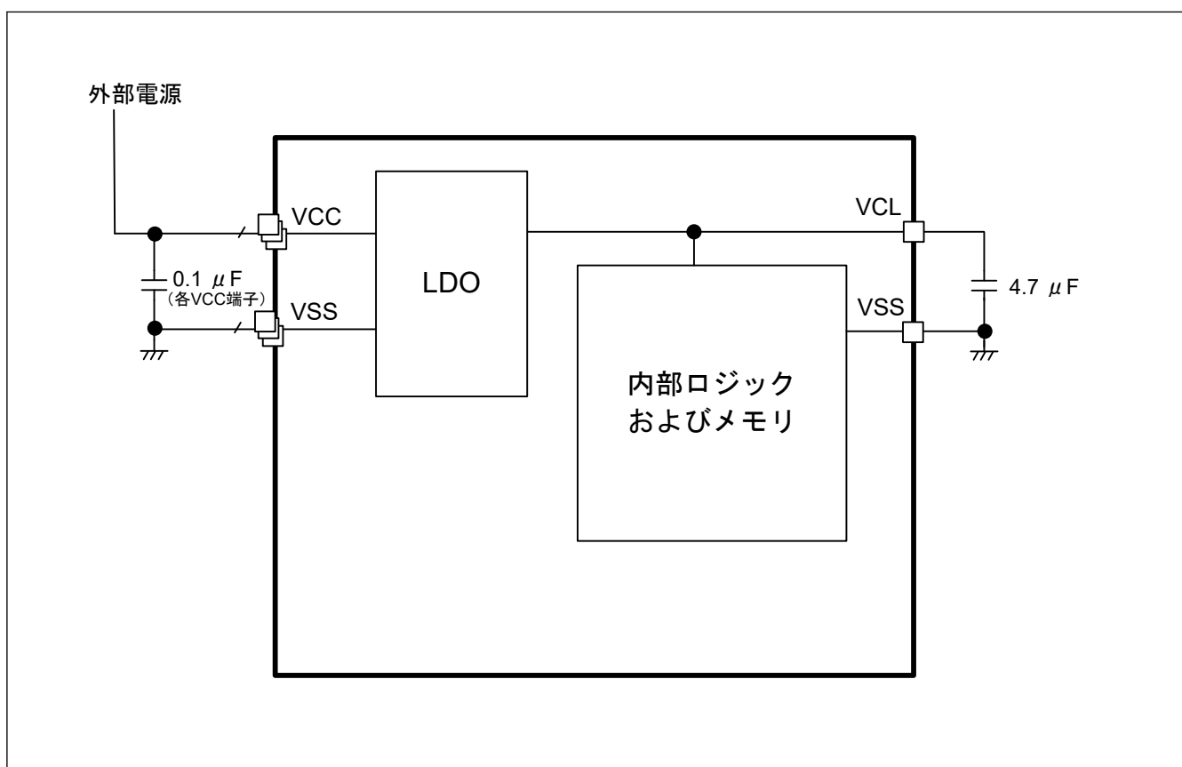
図 38.1 LDO の設定
