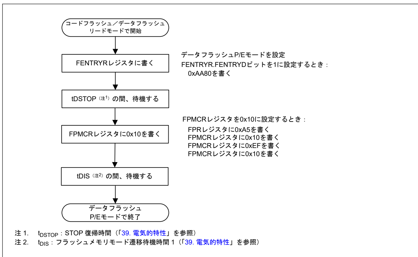
図 35.16 読み出しモードからデータフラッシュ P/E モードへの変更手順
