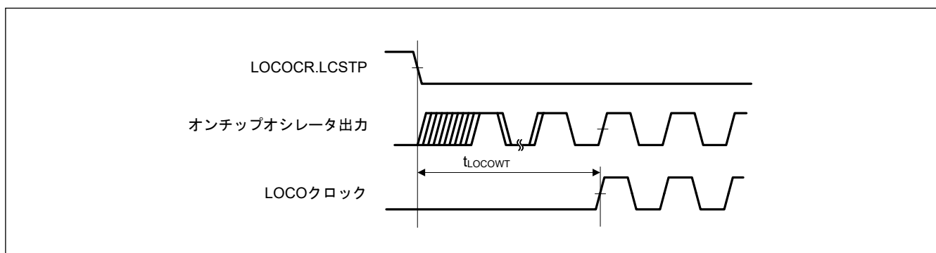
図 50.10 LOCO クロック発振開始タイミング
