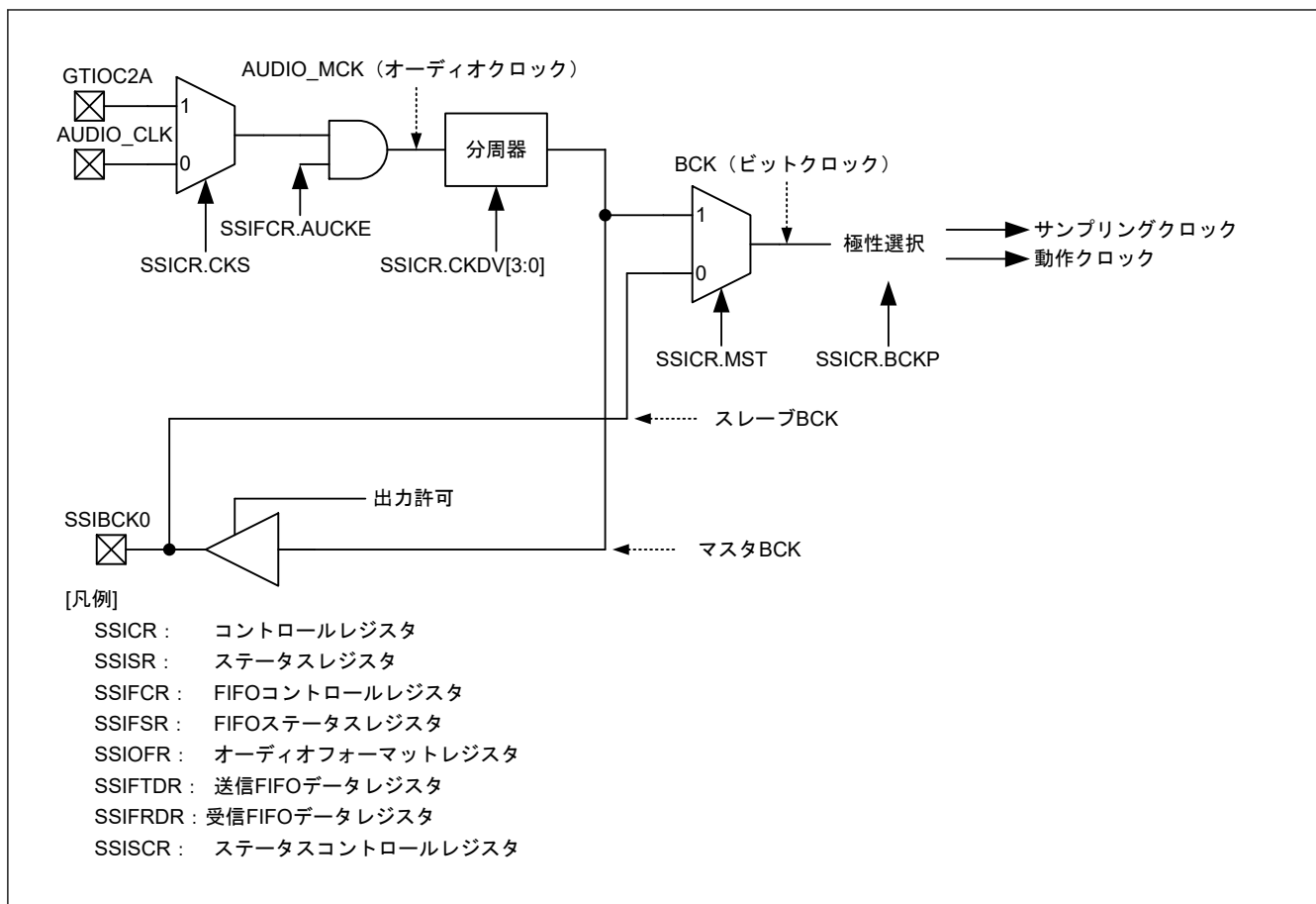
図 35.4 SSIE クロック構成
