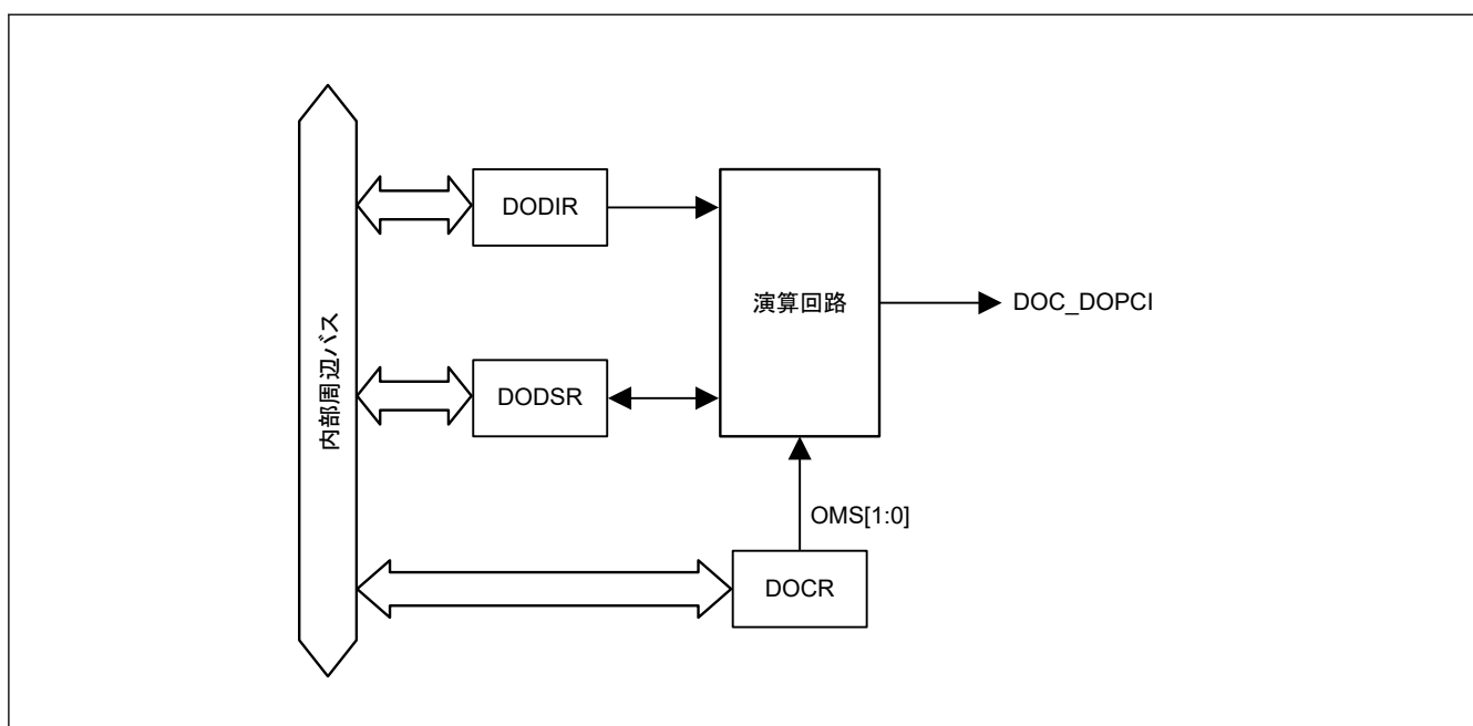
図 44.1 DOC のブロック図
