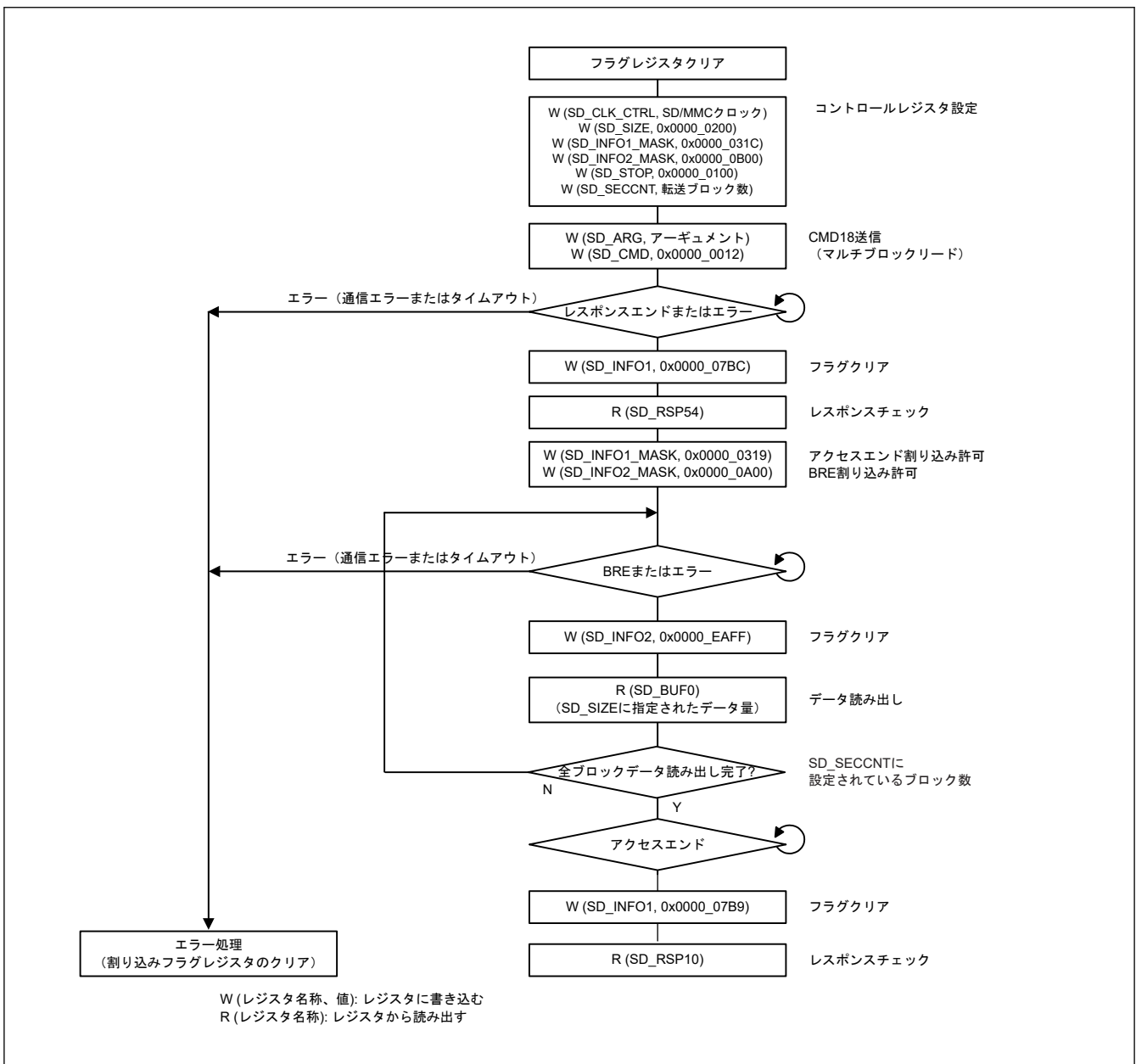
図 36.13 マルチブロックリード動作の例
