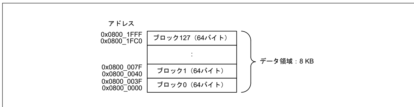
図 47.4 データフラッシュメモリのマップ
