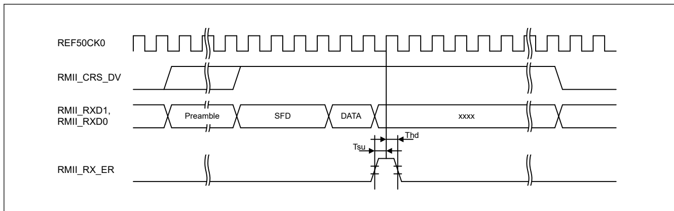
図 50.67 エラー発生時の RMIi 受信タイミング
