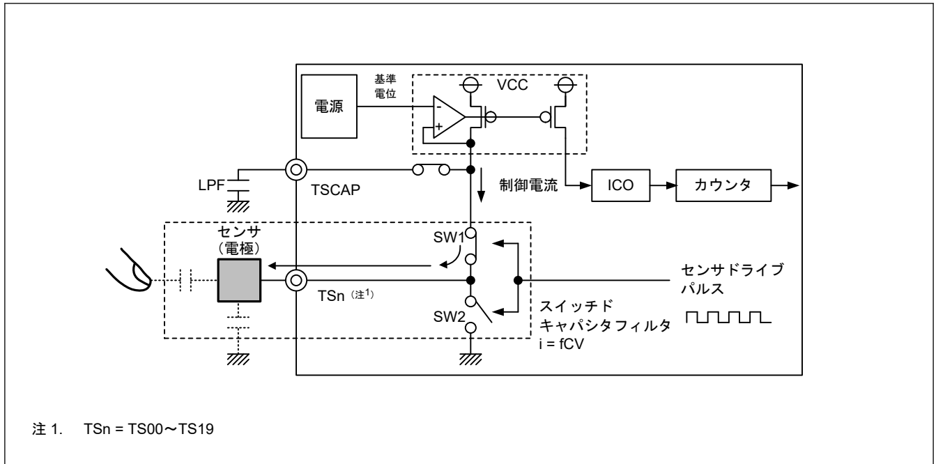
図 43.5 充電動作
