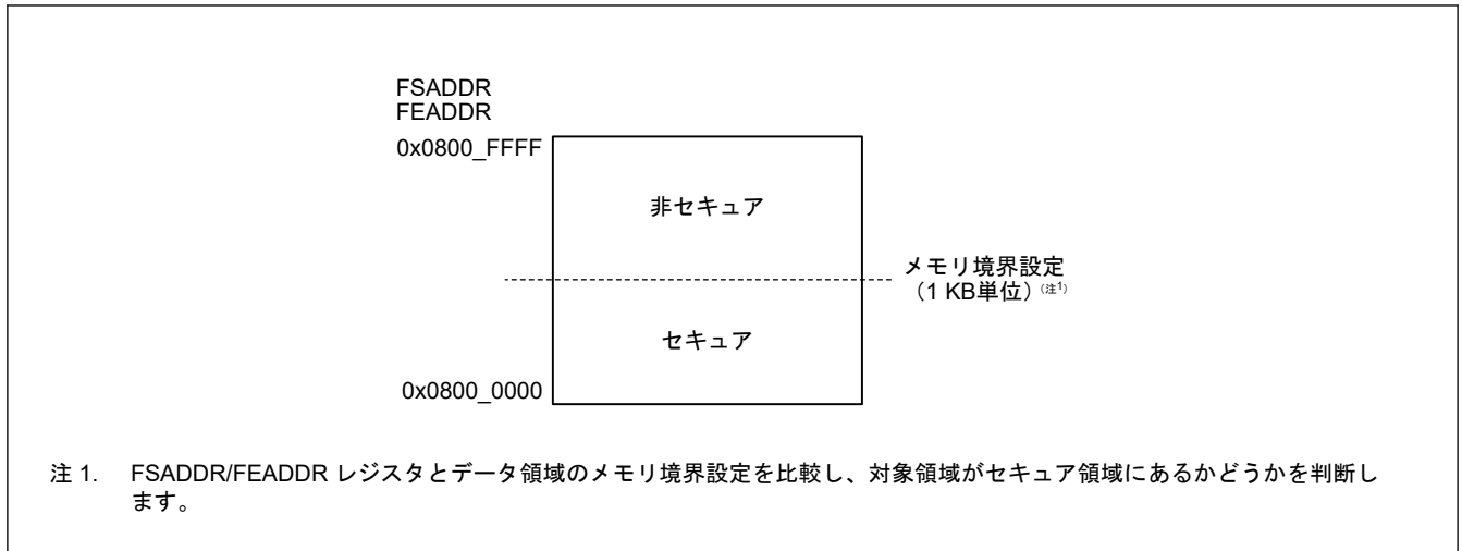
図 47.37 データ領域のセキュア/非セキュア領域
