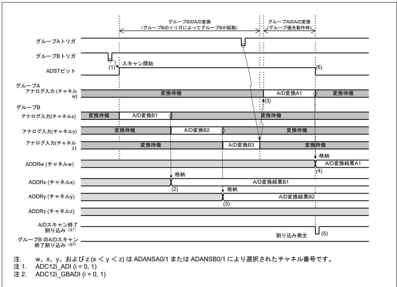
図 40.22 グループ優先動作の例 1-4 : グループ B スキャン中のグループ A トリガ入力、再スキャンなし (ADGSPCR.GBRSCN = 0、ADGSPCR.GBRP = 0、および ADGSPCR.LGRRS = 0 の場合)
