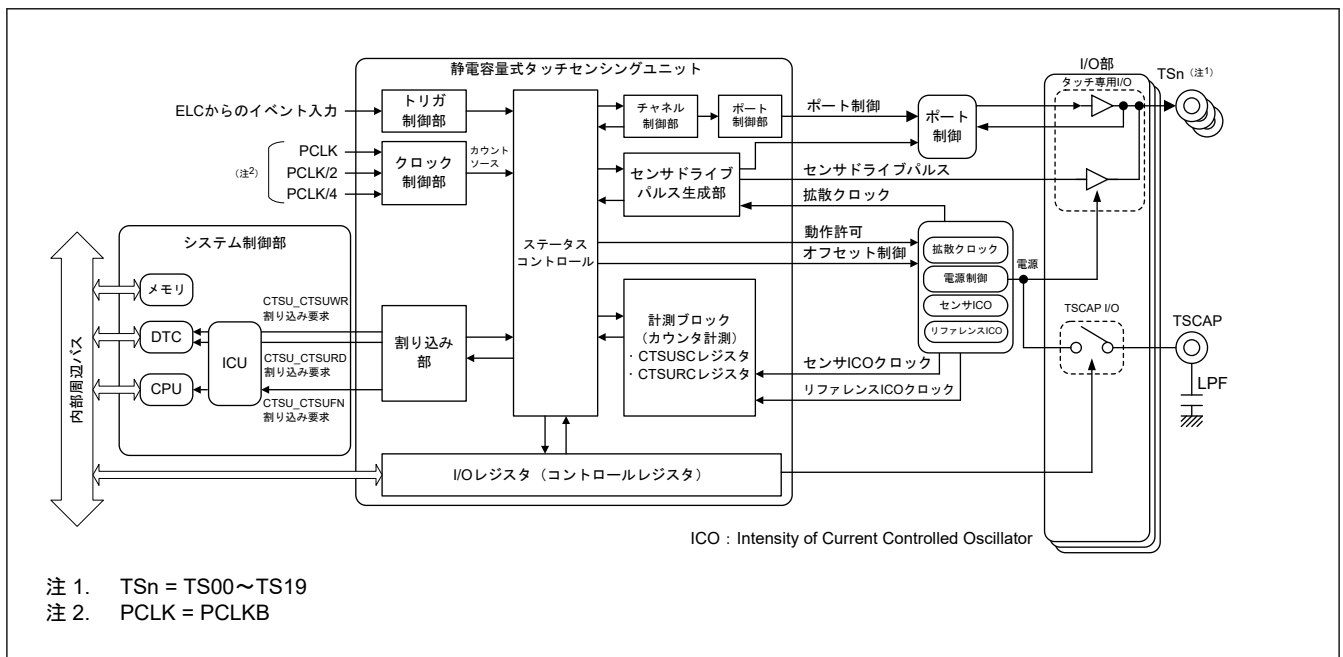
図 43.3 CTSU ブロック図
