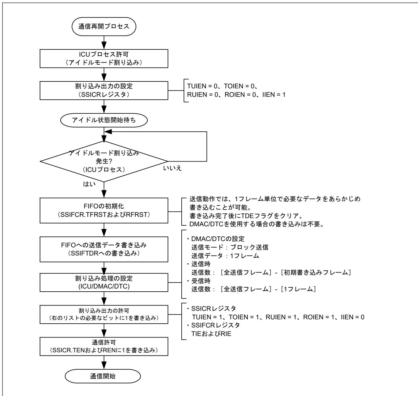
図 35.58 通信再開手順 (CPU 動作手順)
