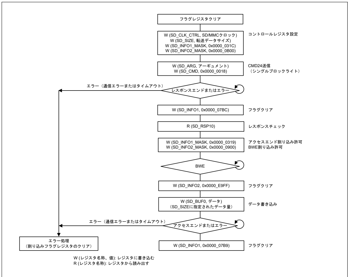
図 36.12 シングルブロックライト動作の例
