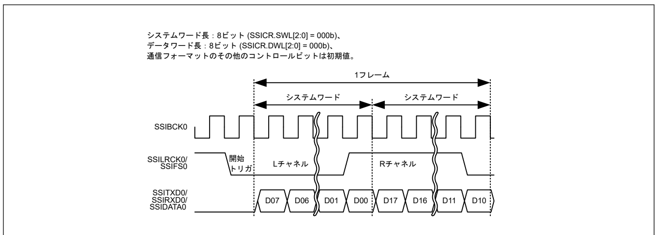
図 35.37 I 2 S フォーマット (パディングなし、システムワード長 = データワード長)
