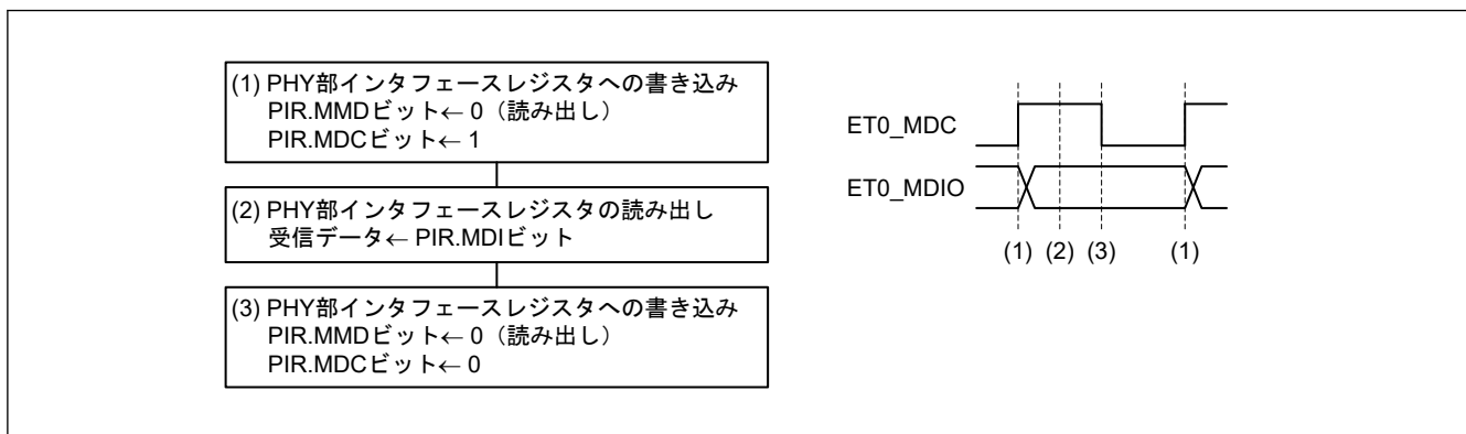
図 26.17 1 ビットデータの読み出しフロー
