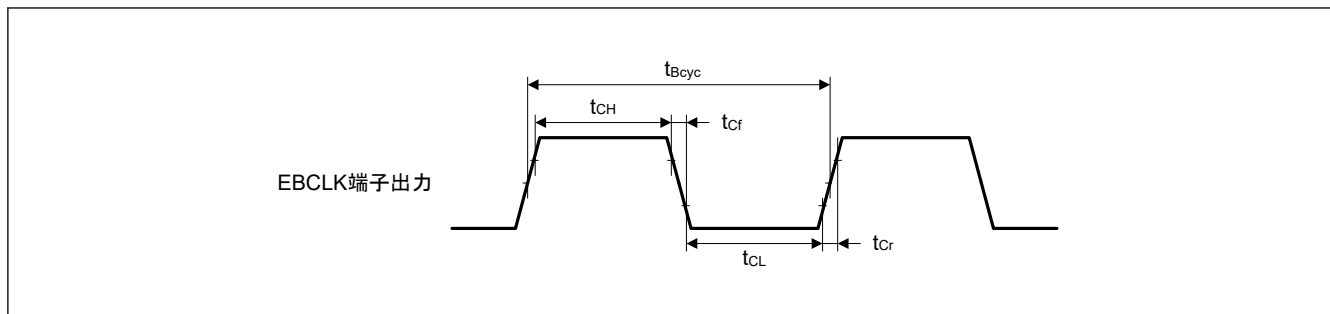
図 50.7 EBCLK 出力タイミング
