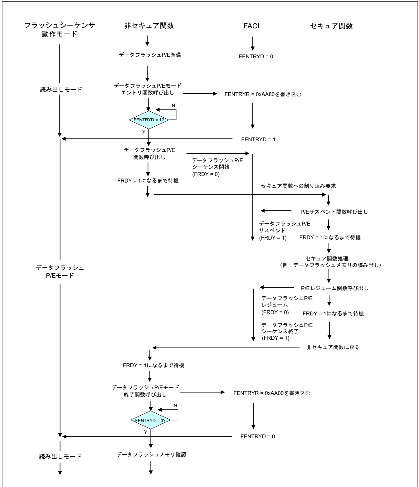
図 47.40 セキュア関数のデータフラッシュ P/E サスペンド例 (P/E 終了を検出するには FRDY ビットを確認)
