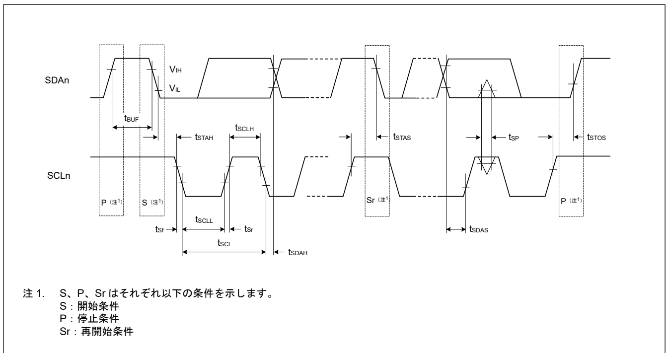
図 50.57 I 2 C バスインタフェース入出力タイミング
