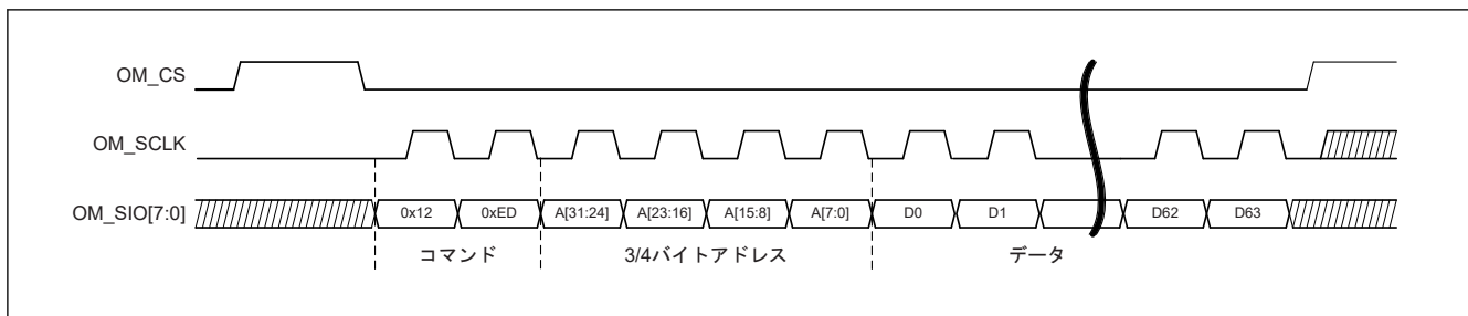
図 34.4 OctaFlash インタフェースでの書き込み動作の波形 (SOPI モード)
