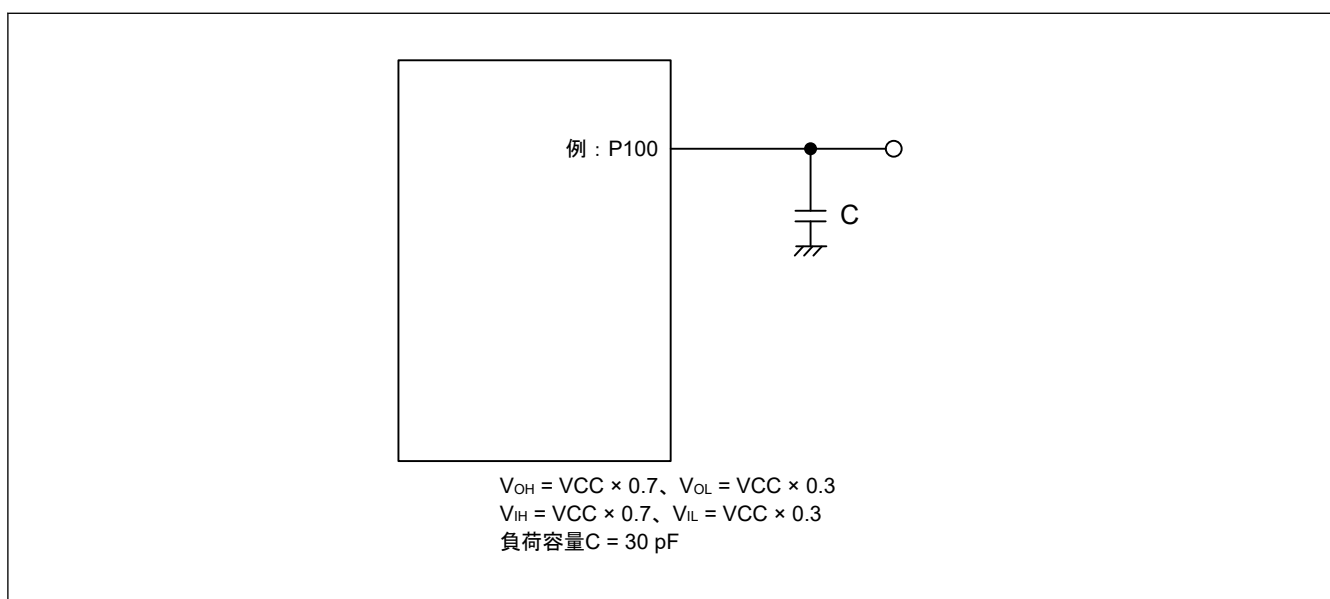
図 50.1 入出力タイミング計測条件
