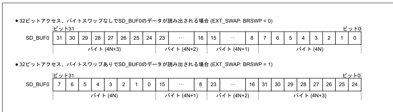
図 36.6 SD_BUF0 からの読み出し
