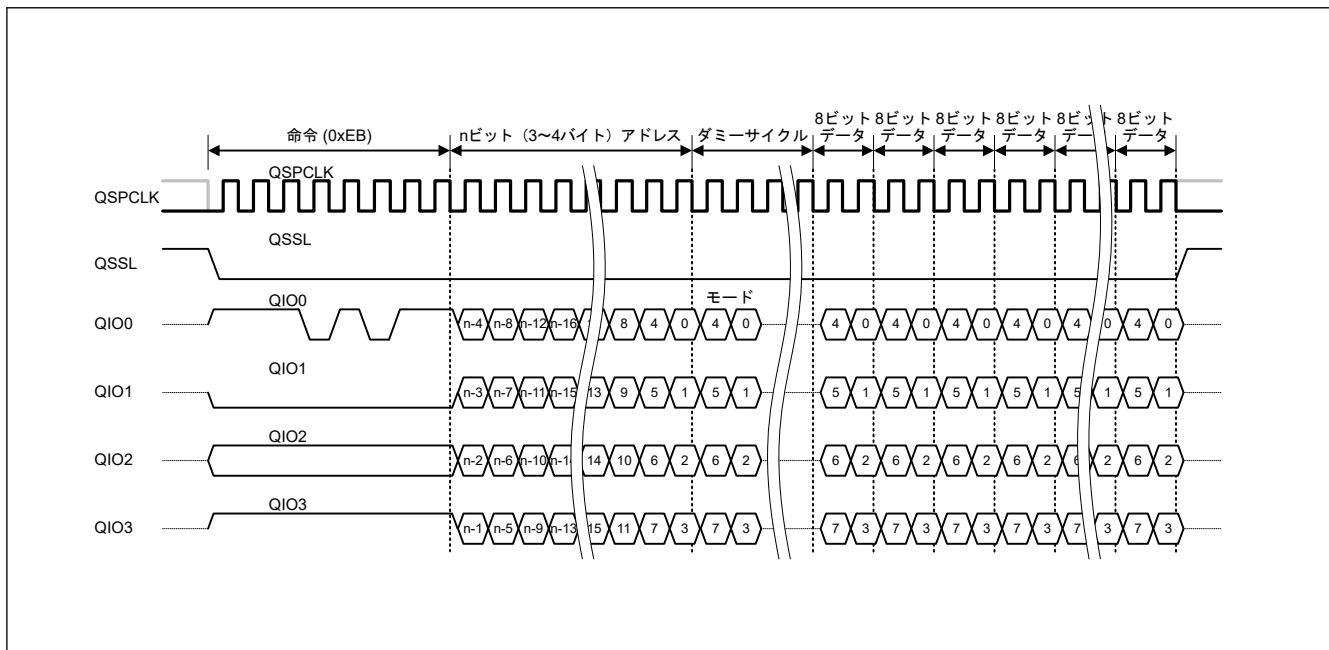
図 33.27 ファストリード Quad I/O パスサイクル
