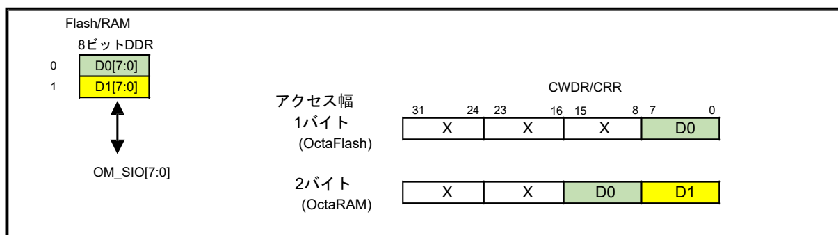
図 34.12 OctaFlash および OctaRAM スペースの構成レジスタデータアラインメント
