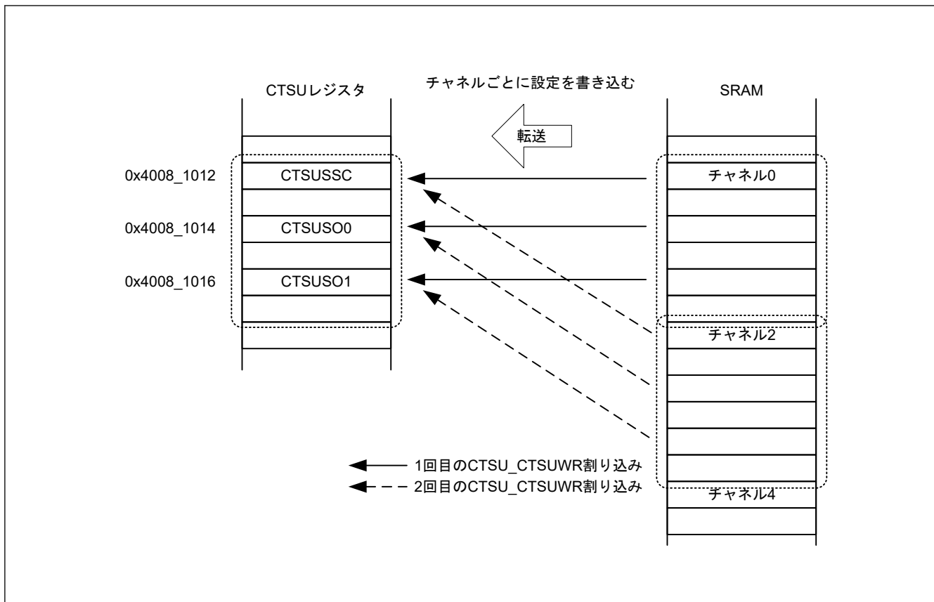
図 43.19 CTSU_CTSUWR 割り込みを用いた DTC 転送動作例
