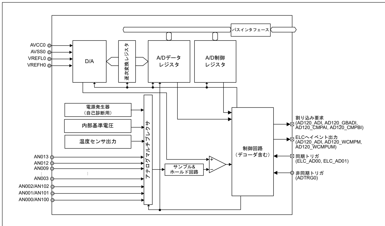
図 40.1 ADC12 のブロック図 (ユニット 0)
