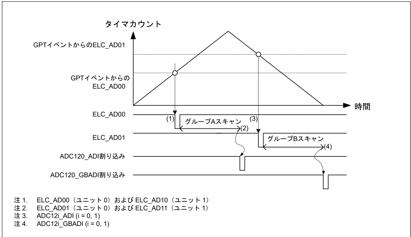
図 40.16 グループスキャンモードの基本動作例 (ELC からの同期トリガ使用)
