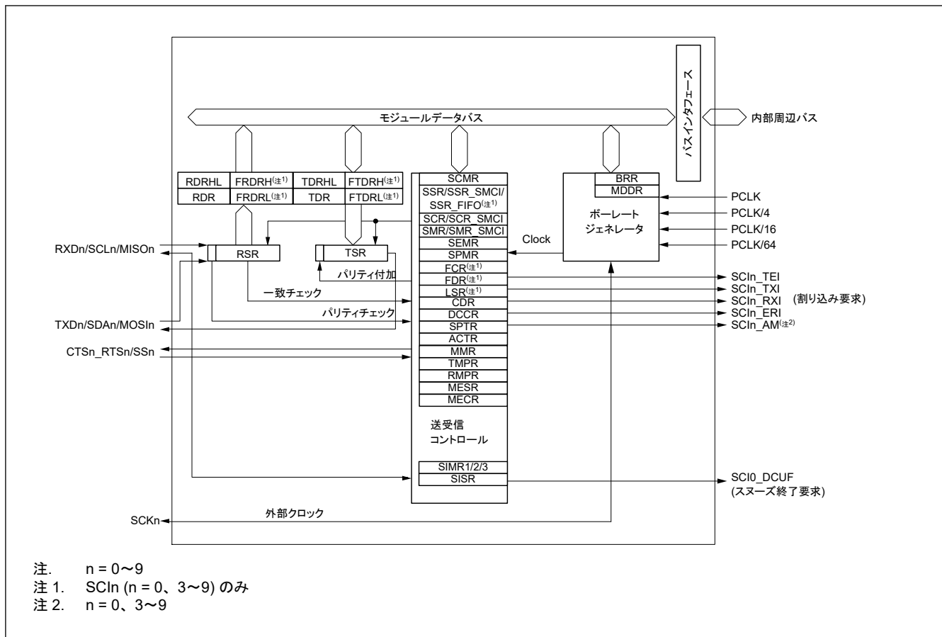
図 29.1 SCI のブロック図
