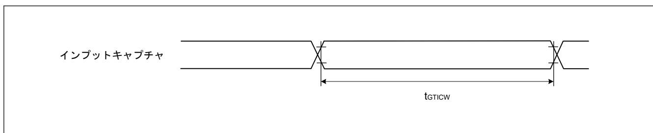
図 50.29 GPT インพุットキャプチャタイミング
