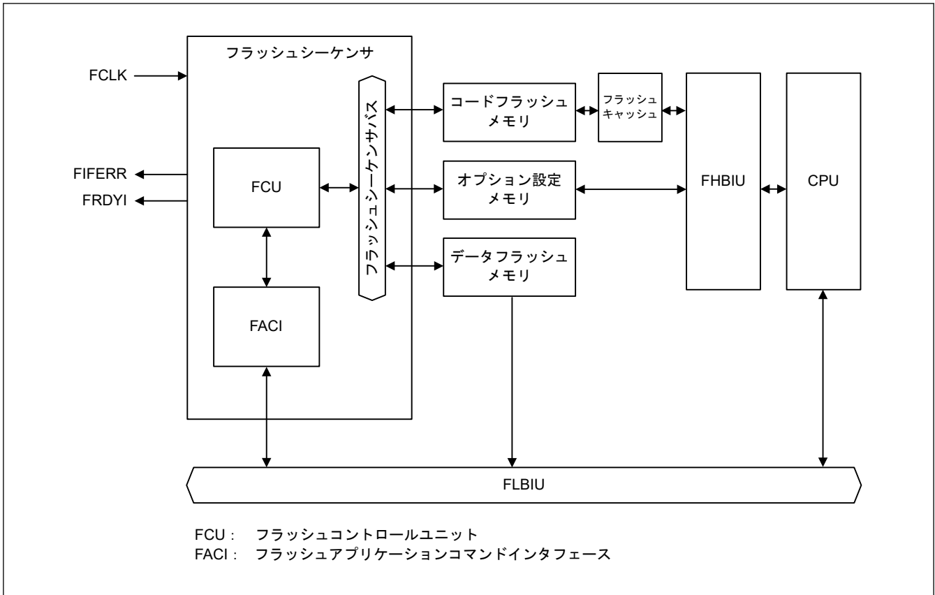
図 47.1 フラッシュメモリ関連モジュールのブロック図
