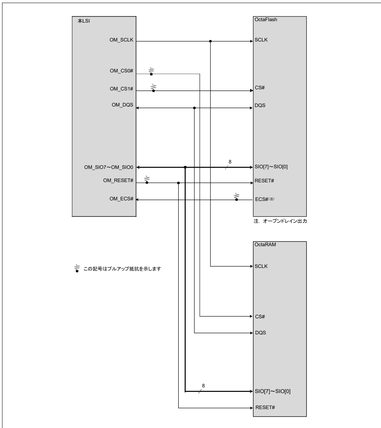
図 34.2 OSPI と OctaFlash および OctaRAM デバイスとの接続の例
