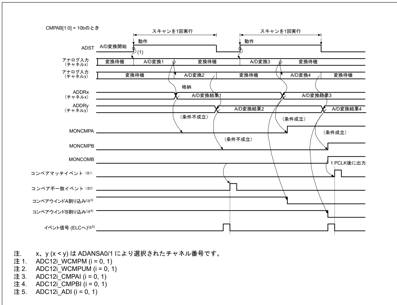
図 40.30 コンペア機能のイベント出力の動作例（アナログ入力（チャンネル x、y）を比較）
