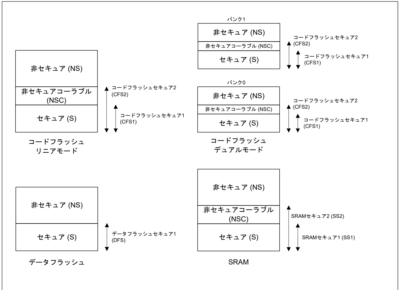
図 49.1 メモリマッピング
