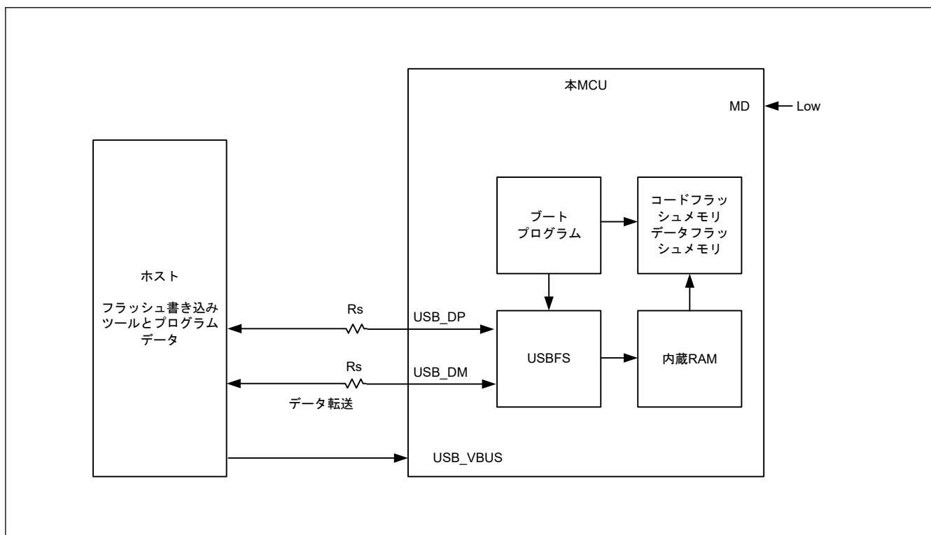
図 47.44 ブートモード (USB インタフェース) のシステム構成図
