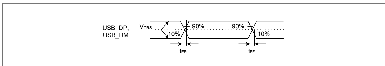
図 50.76 フルスピードモードにおける USB_DP、USB_DM の出力タイミング
