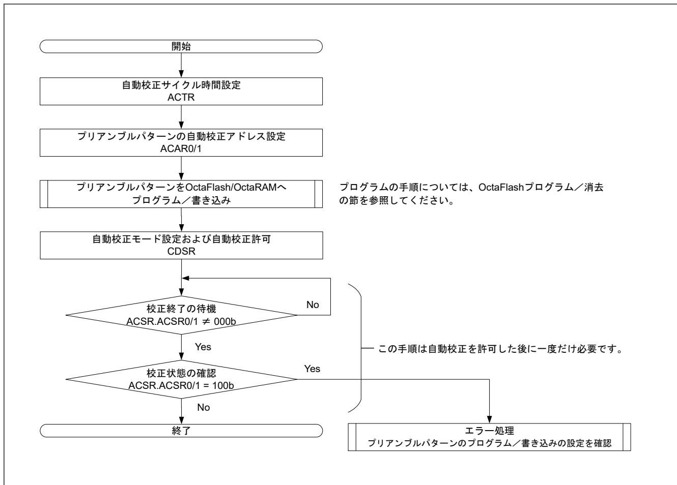
図 34.14 自動校正設定フロー
