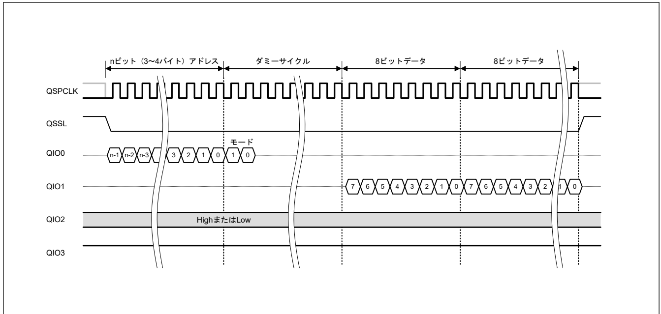
図 33.20 XIP モード時のファストリードパスサイクル
