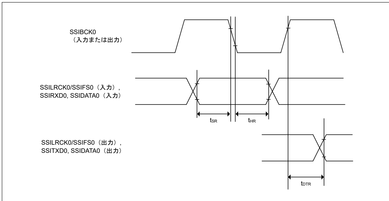
図 50.61 SSICR.BCKP = 1 の場合の SSIE データ送受信タイミング
