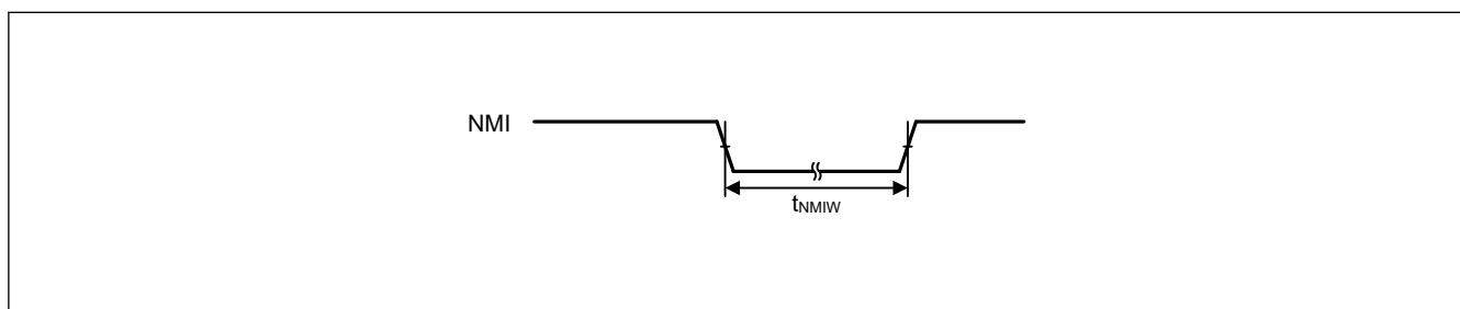
図 50.18 NMI 割り込み入カタイミング
