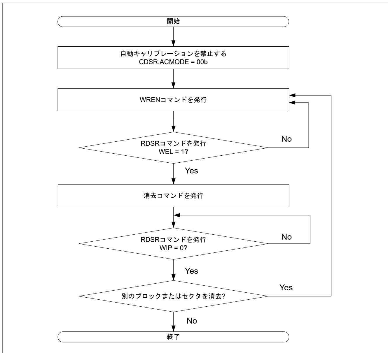
図 34.18 OctaFlash 消去の手順
