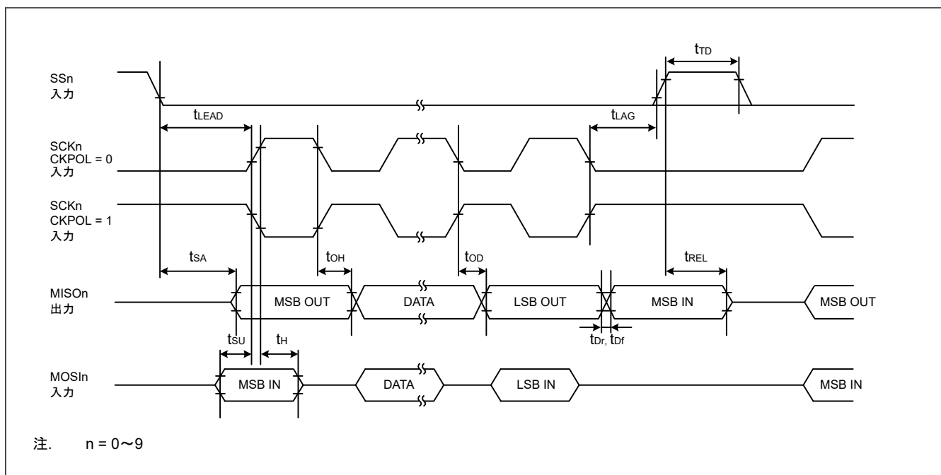
図 50.39 CKPH = 1 の場合におけるスレーブの SCI 簡易 SPI モードタイミング
