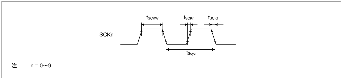
図 50.34 SCK クロック入出力タイミング
