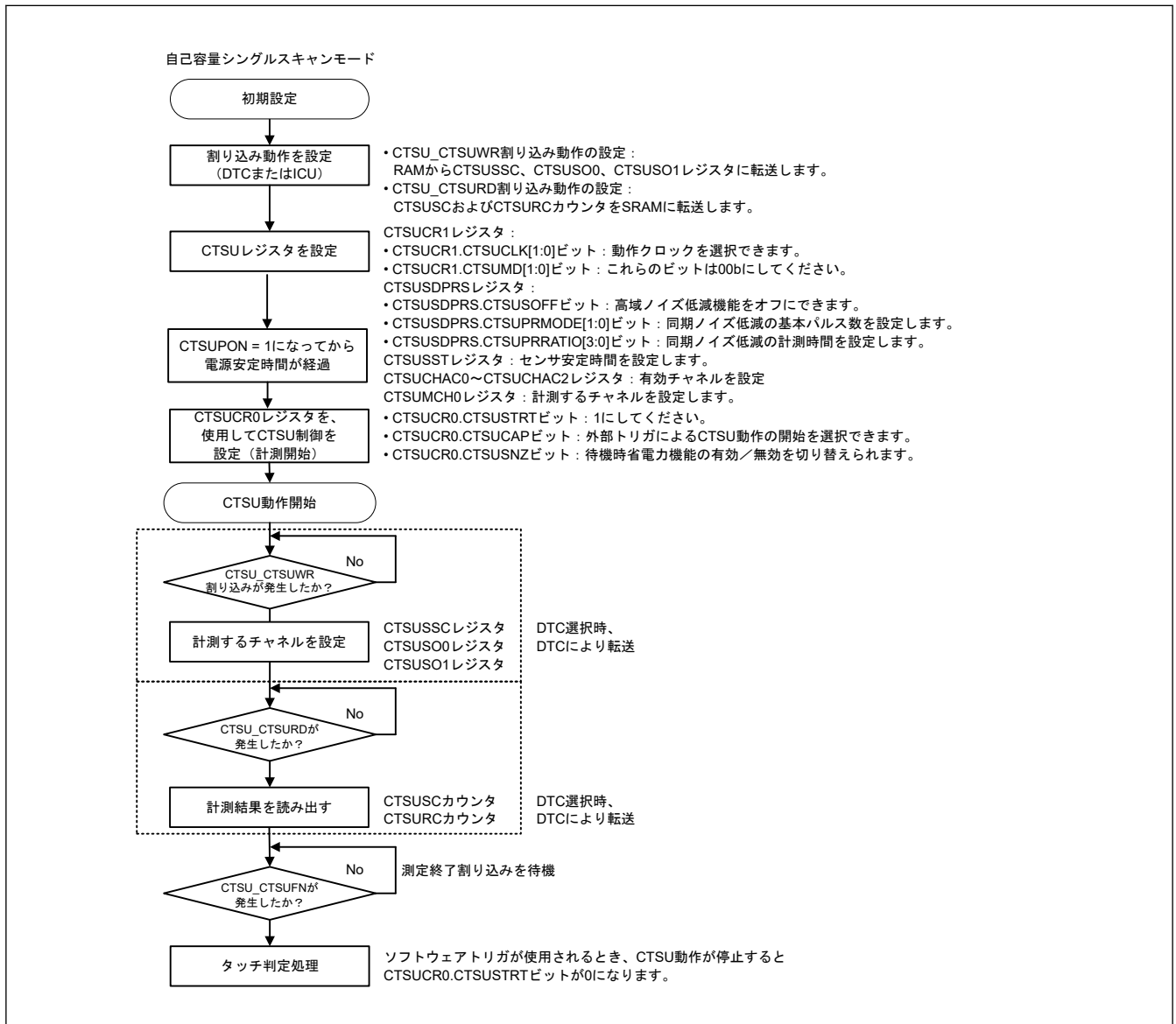
図 43.12 自己容量シングルスキャンモードのソフトウェアフローと動作例
