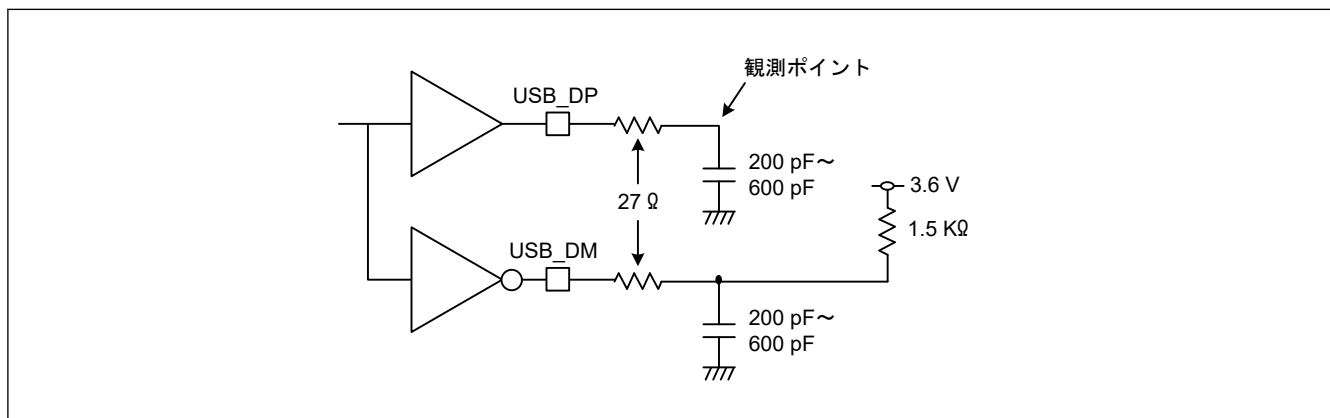
図 50.75 Low-speed モードにおける測定回路
