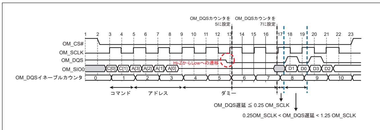
図 34.22 OM_DQS クロック入力が Hi-Z から Low に遷移するタイミングの例 (フラッシュ DOPI モード、ダミーサイクル数 = 4、OM_DQS プレサイクル ON)
