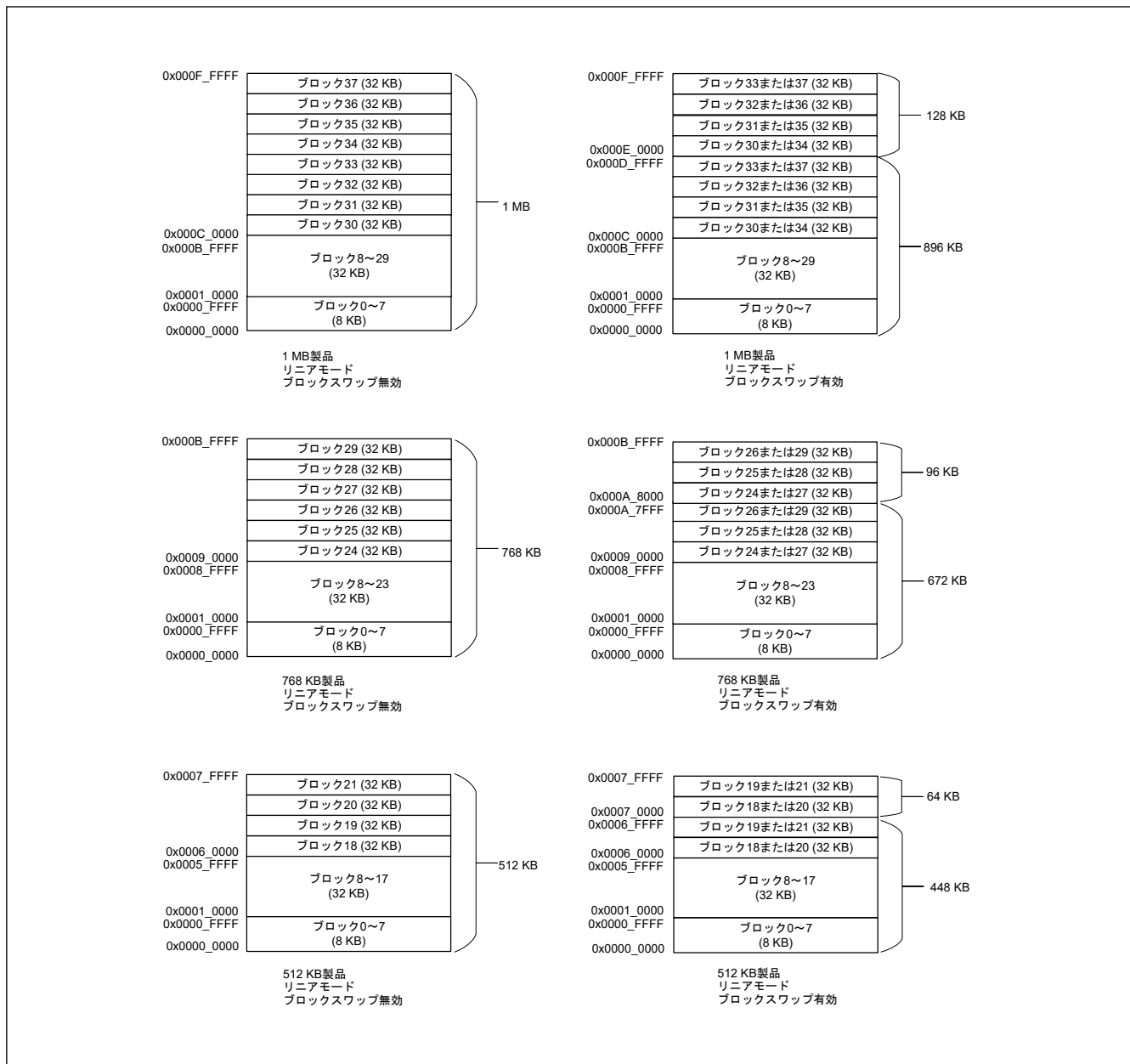
図 6.2 リニアモード時のフラッシュメモリのマッピング
