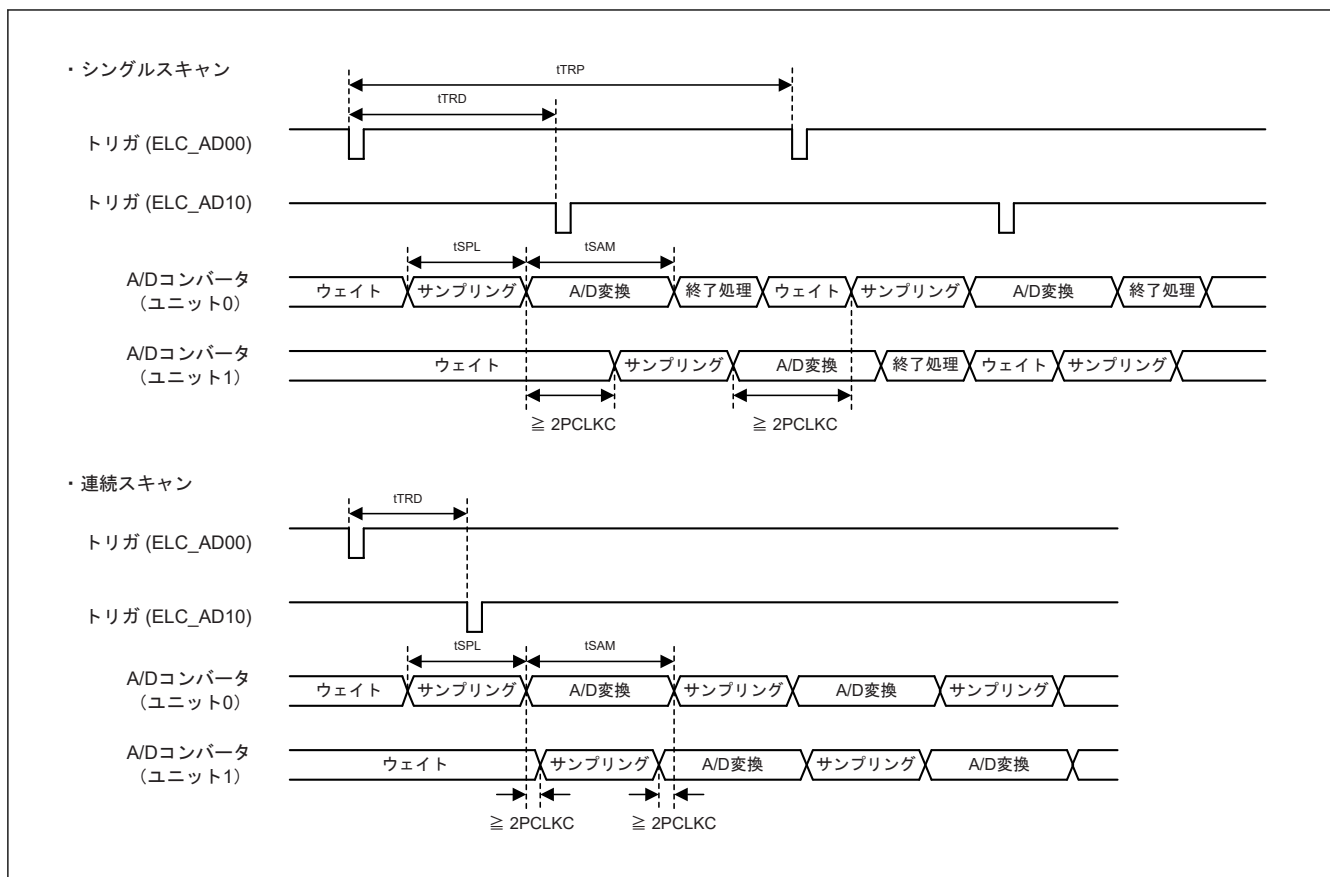
図 40.24 インターリーブ動作におけるトリガ入力タイミング
