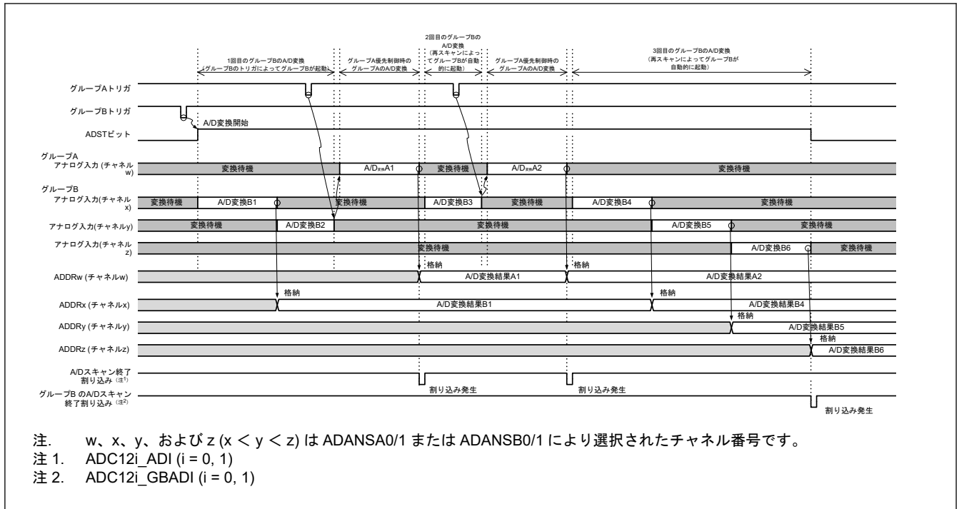
図 40.20 グループ優先動作の例 1-2 : グループ B 再スキャン中のグループ A トリガ入力、再スキャンあり (ADGSPCR.GBRSCN = 1, ADGSPCR.GBRP = 0, および ADGSPCR.LGRRS = 0 の場合)
