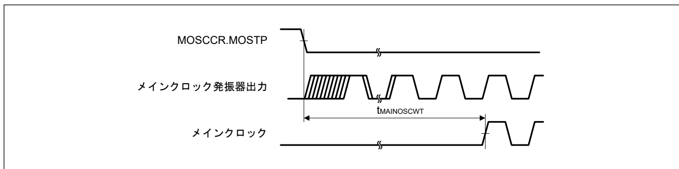
図 50.9 メインクロック発振開始タイミング
