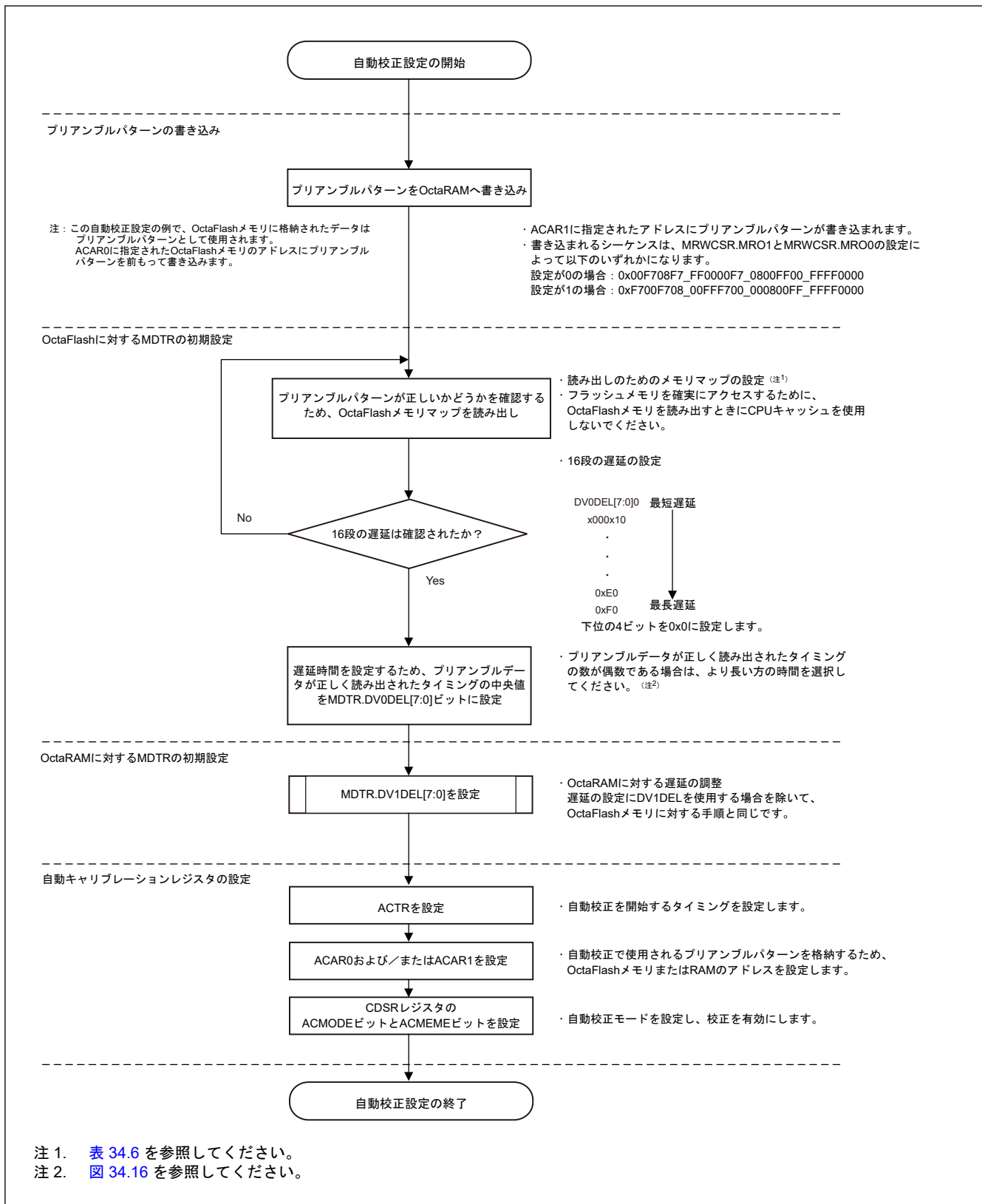
図 34.15 手動校正フローを用いた自動校正設定
