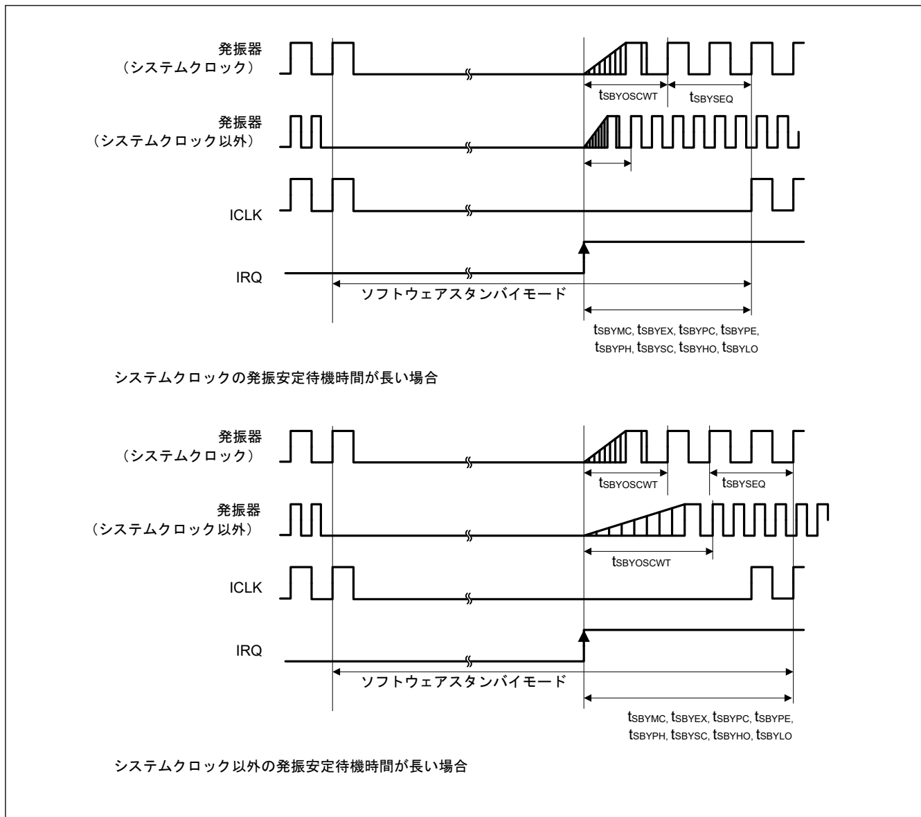
図 50.15 ソフトウェアスタンバイモード解除タイミング
