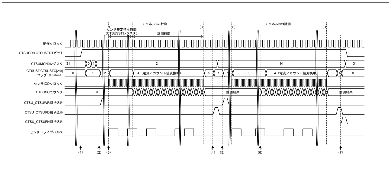
図 43.15 自己容量マルチスキャンモードのタイミング (計測開始条件がソフトウェアトリガの場合)
