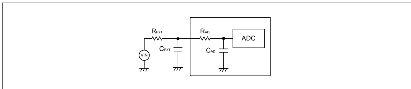
図 40.40 サンプル&ホールド回路の簡略図
