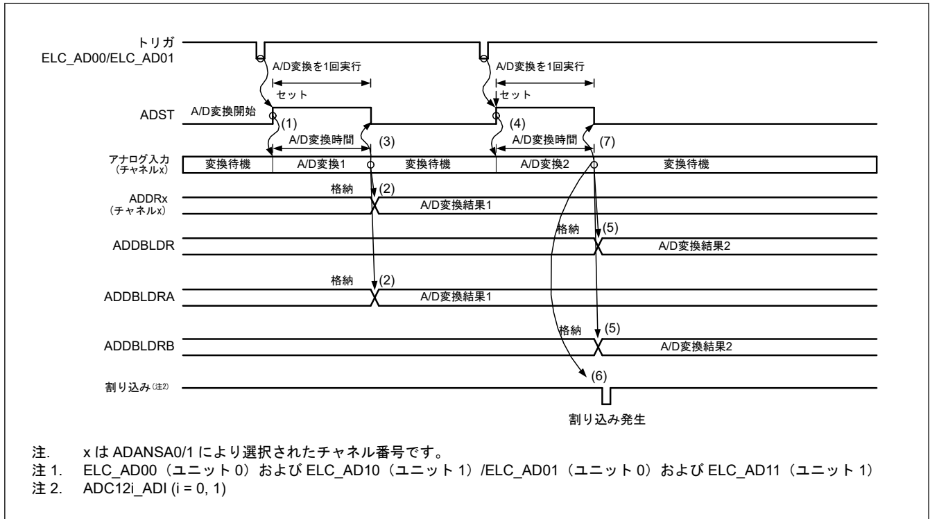
図 40.12 アナログ入力 (チャンネル x) と ELC_AD00 (ユニット 0) および ELC_AD10 (ユニット 1) /ELC_AD01 (ユニット 0) および ELC_AD11 (ユニット 1) の重複選択時のダブルトリガモード拡張動作例
