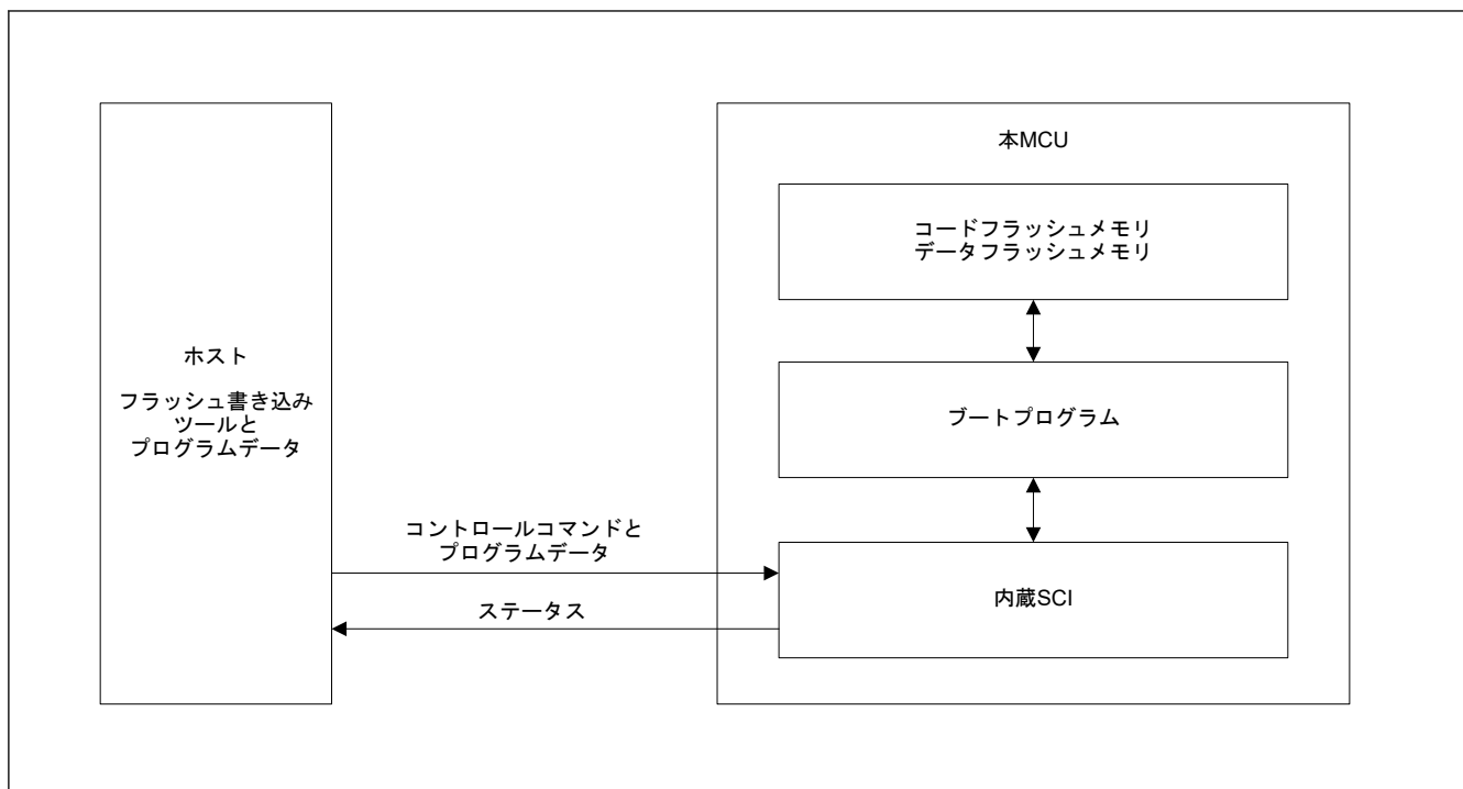
図 47.43 ブートモード (SCI インタフェース) 時のシステム構成
