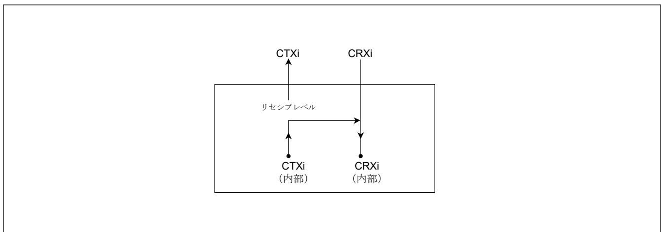
図 31.6 リッスンオンリーモード選択時の接続 (i = 0, 1)
