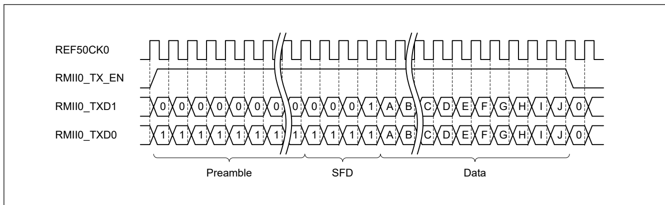
図 26.12 RMII フレーム送信タイミング (正常送信時)
