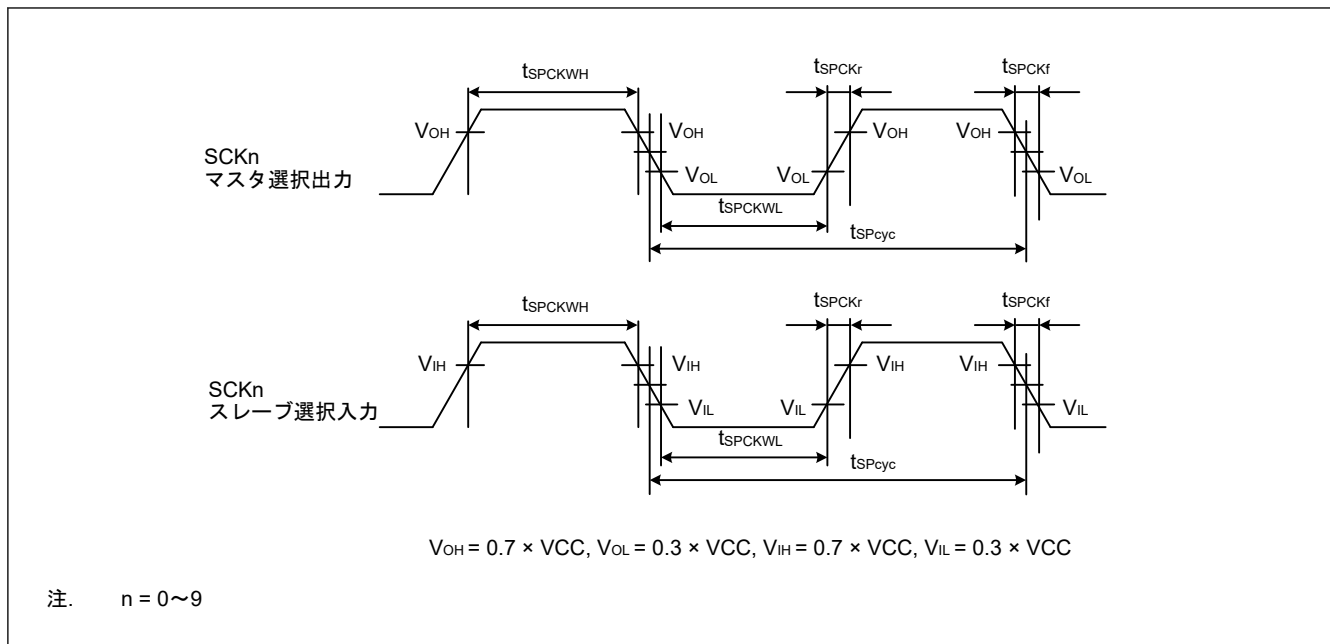
図 50.36 SCI 簡易 SPI モードクロックタイミング
