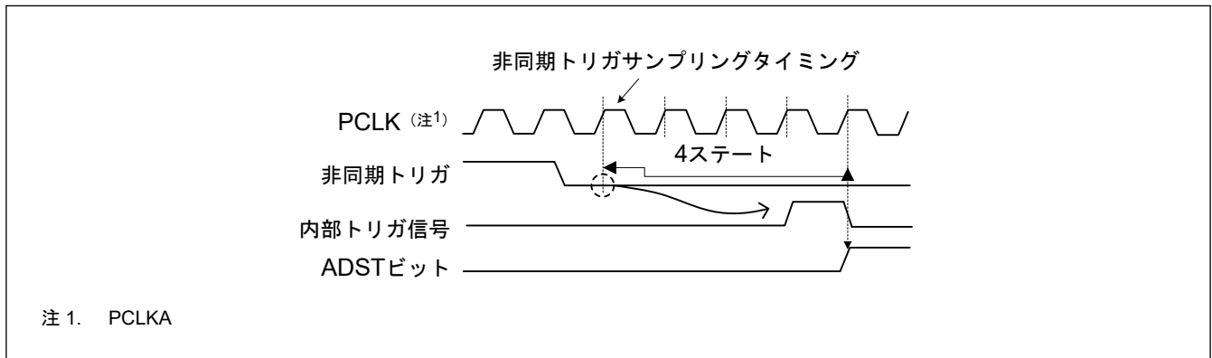
図 40.36 非同期トリガ入力タイミング
