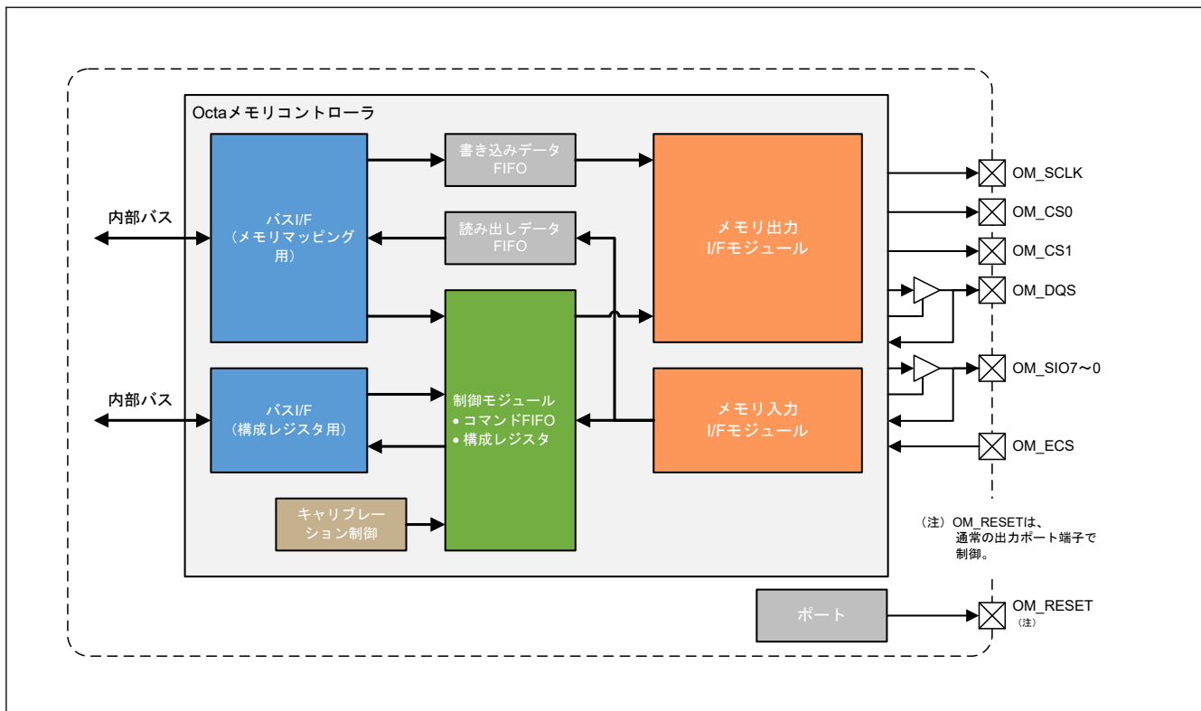
図 34.1 ブロック図
