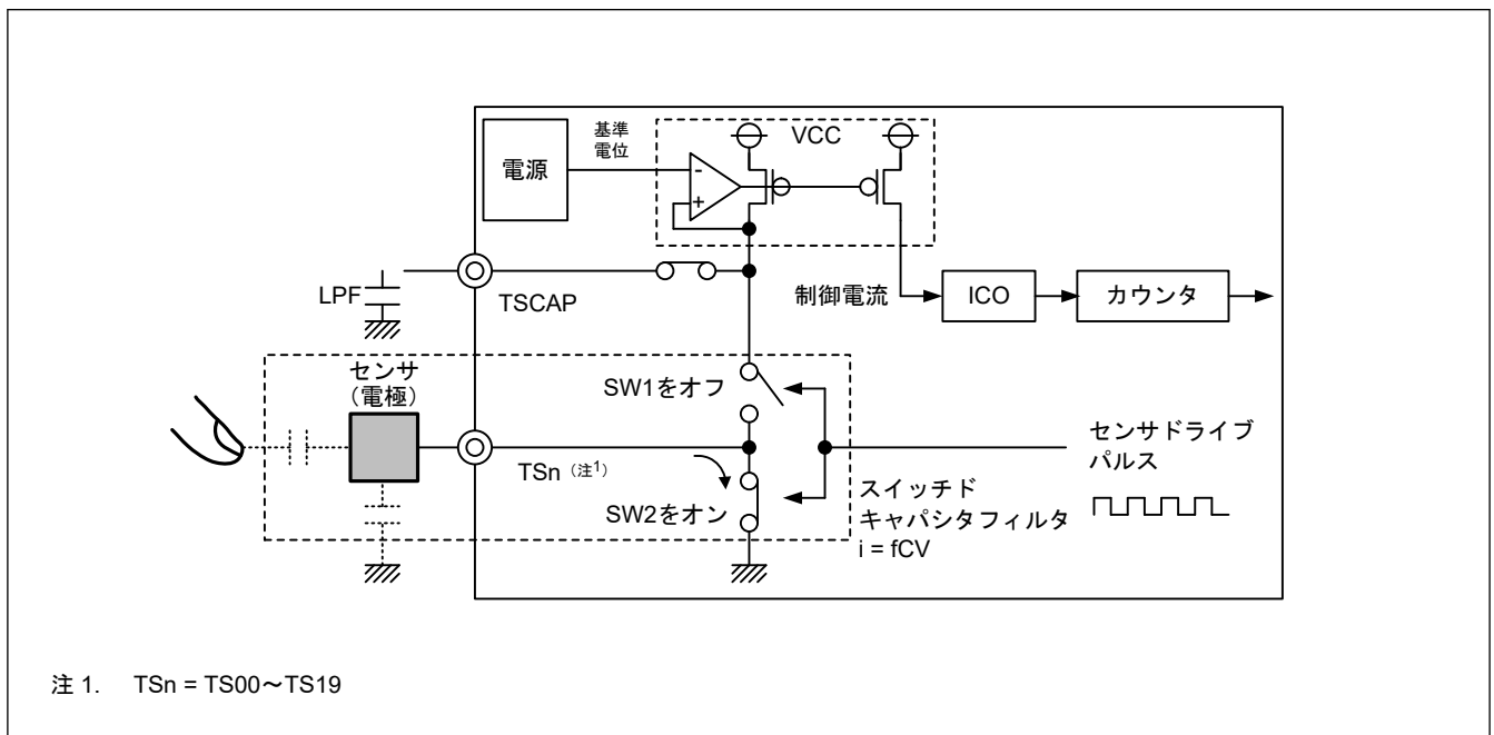
図 43.6 放電動作
