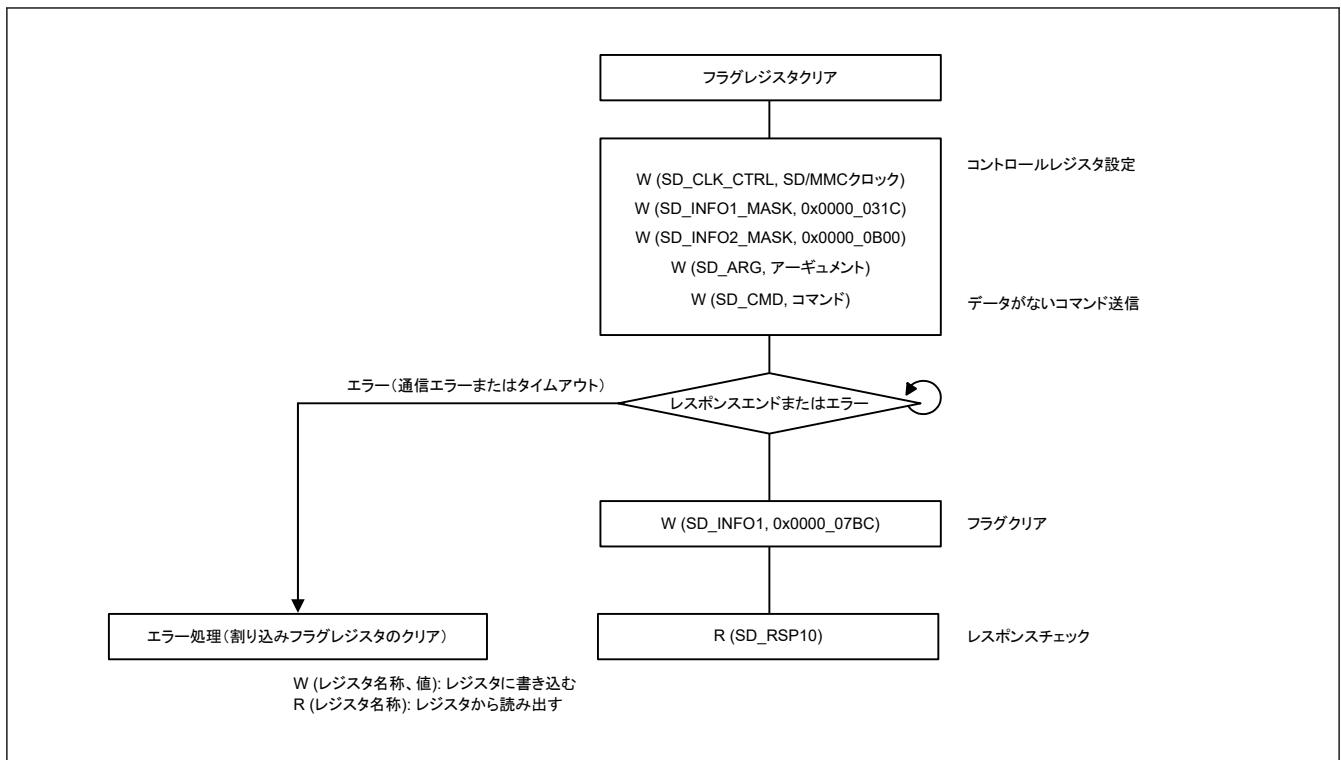
図 36.10 データがないコマンドのフロー例
