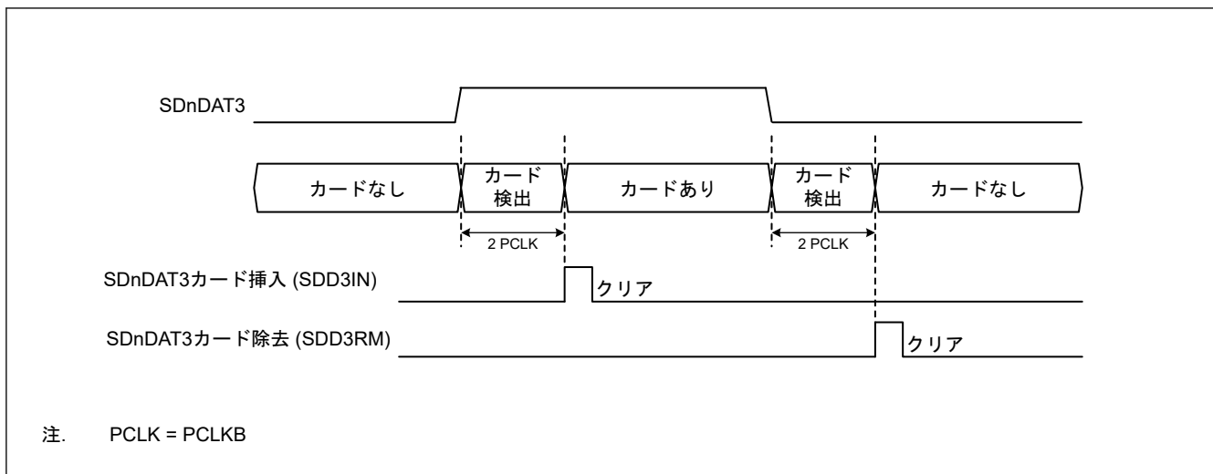
図 36.8 SDnDAT3 による SD カード検出
