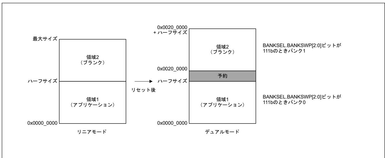
図 47.47 リニアモードでのデュアルモード用アプリケーションの書き込み
