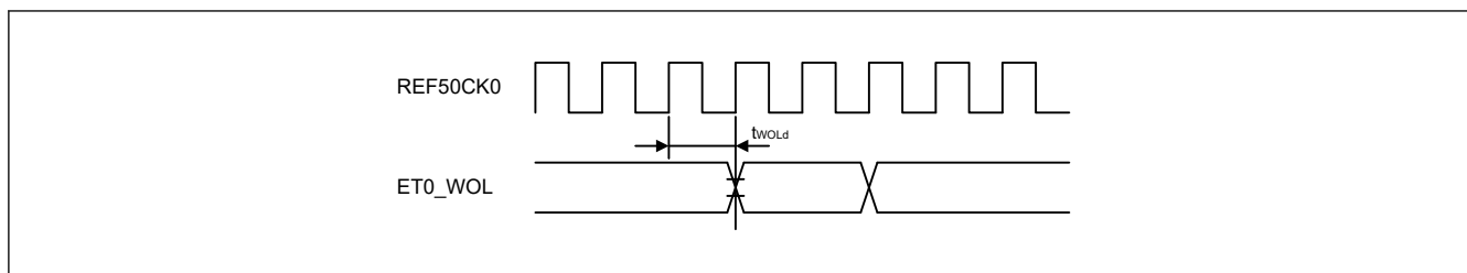
図 50.68 RMIi に対する WOL 出力タイミング
