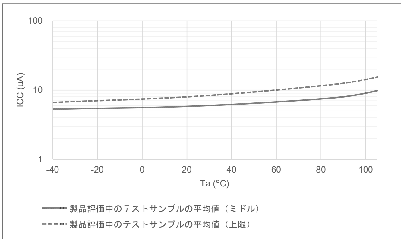
図 50.5 ディープソフトウェアスタンバイモード時の温度依存性、SRAM および USB レジューム検出部への電源供給なし、パワーオンリセット回路、低消費電力機能有効（参考データ）
