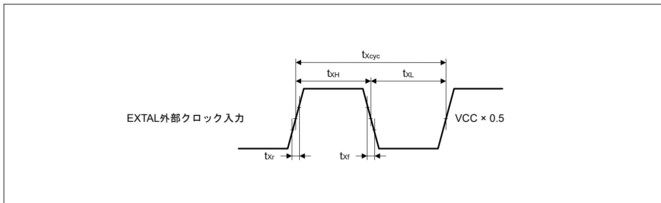
図 50.8 EXTAL 外部クロック入力タイミング
