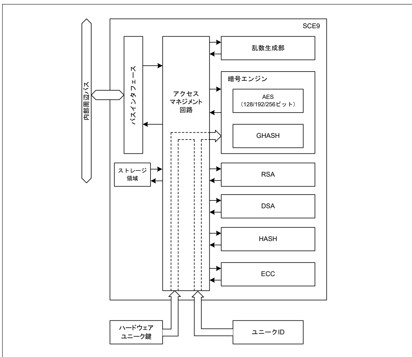
図 39.1 SCE9 のブロック図
