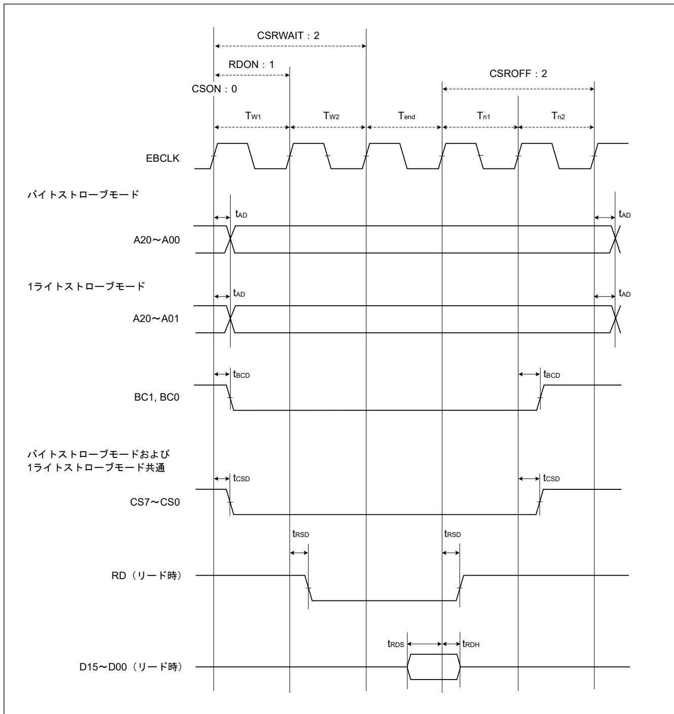
図 50.22 バスクロック同期を使用したノーマルリードサイクルの外部バスタイミング
