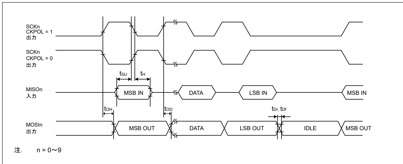
図 50.38 CKPH = 0 の場合におけるマスタの SCI 簡易 SPI モードタイミング
