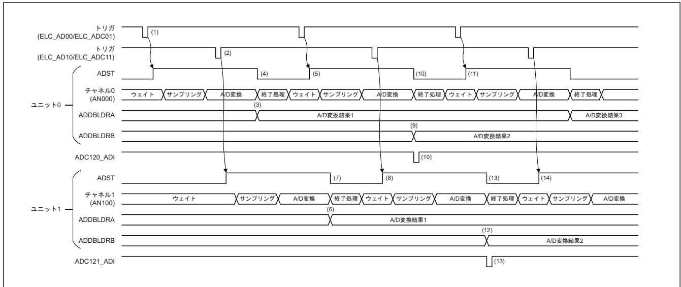
図 40.27 シングルスキャンモードの動作例（ダブルトリガ拡張モード選択、AN000 および AN100 選択、インターリーブ動作）
