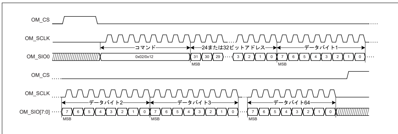
図 34.3 OctaFlash インタフェースでの書き込み動作の波形 (SPI モード)
