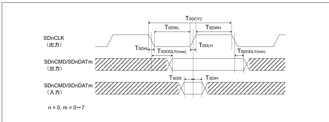
図 50.63 SD/MMC ホストインタフェース信号タイミング
