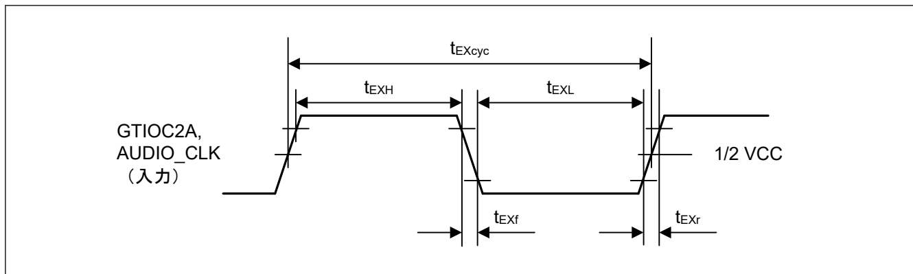
図 50.59 クロック入力タイミング
