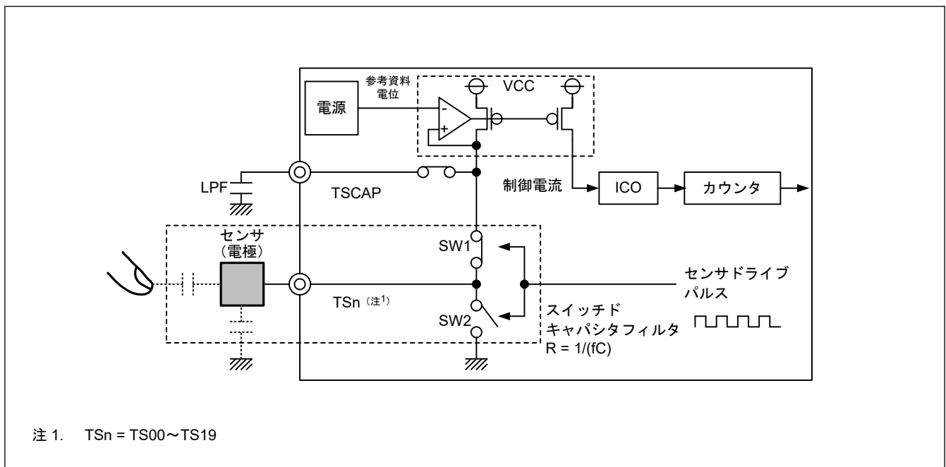
図 43.4 計測部回路
