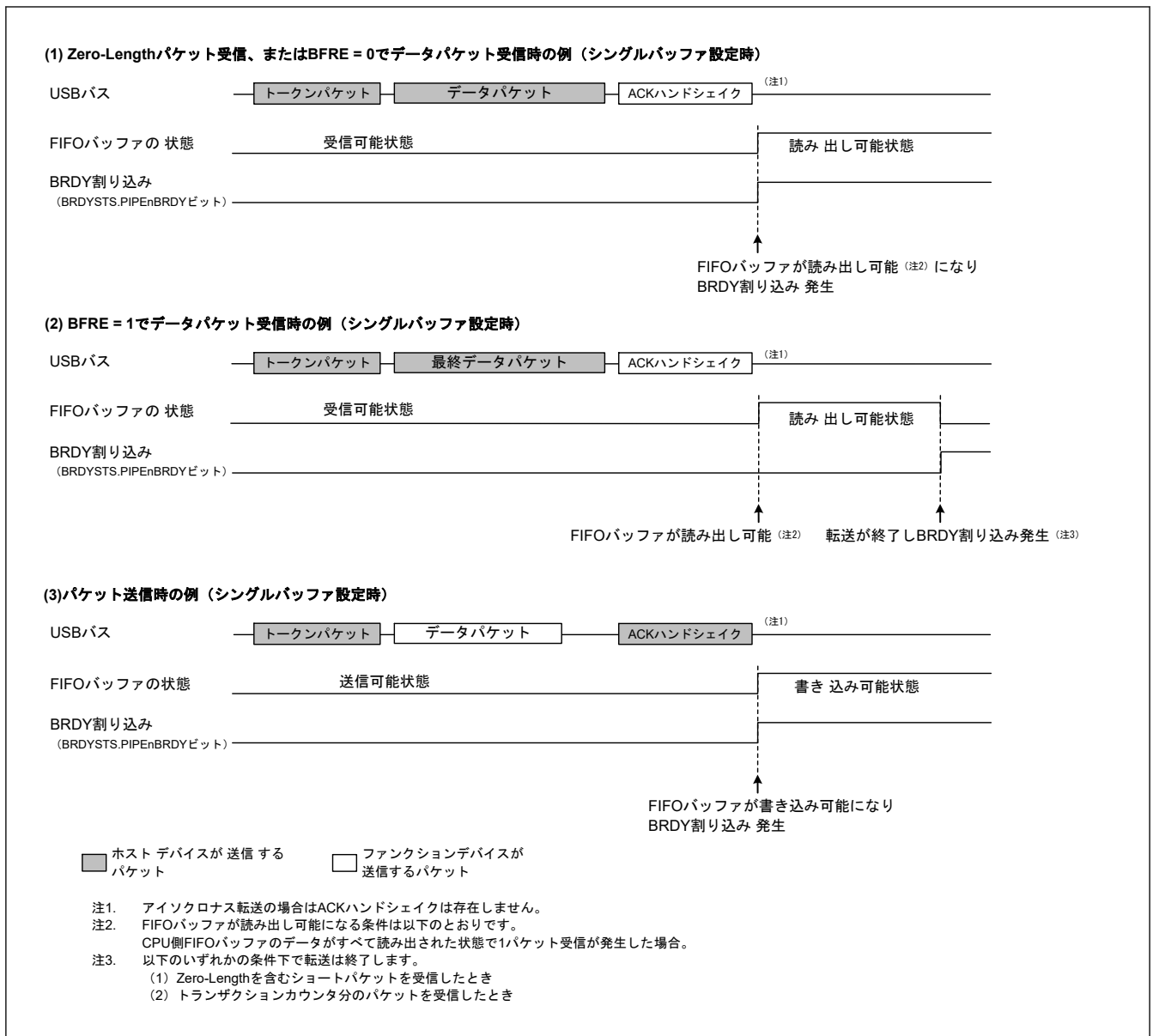
図 28.12 BRDY 割り込み発生タイミング
