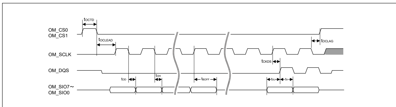
図 50.53 SOPI 転送フォーマット送受信タイミング
