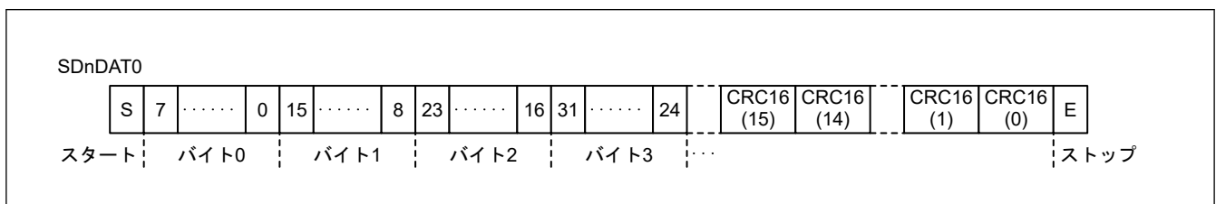
図 36.2 1 ビット幅モードの SDnDAT
