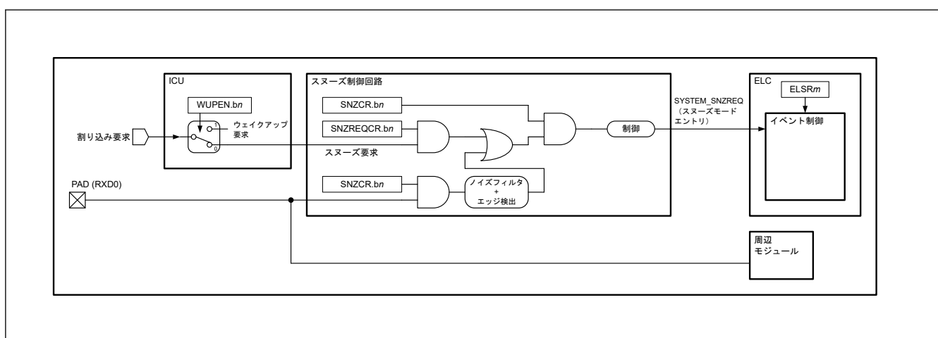
図 10.3 スヌーズモードへの遷移時構成
