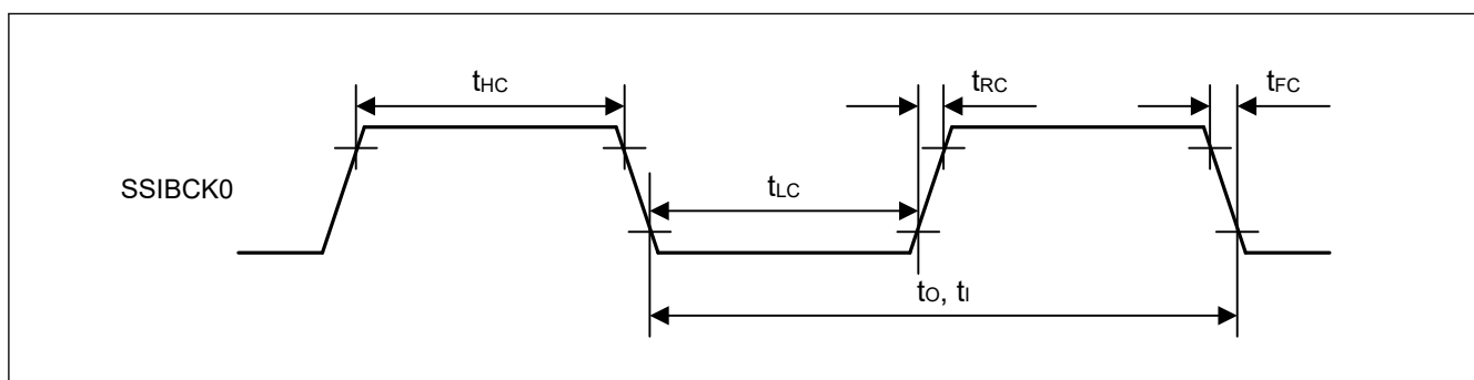
図 50.58 SSIE クロック入出力タイミング
