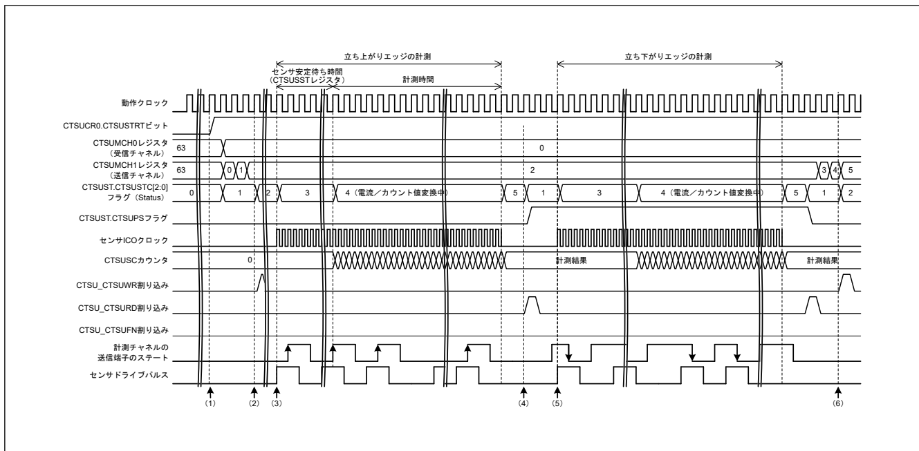
図 43.17 相互容量フルスキャンモードのタイミング (計測開始条件がソフトウェアトリガの場合)
