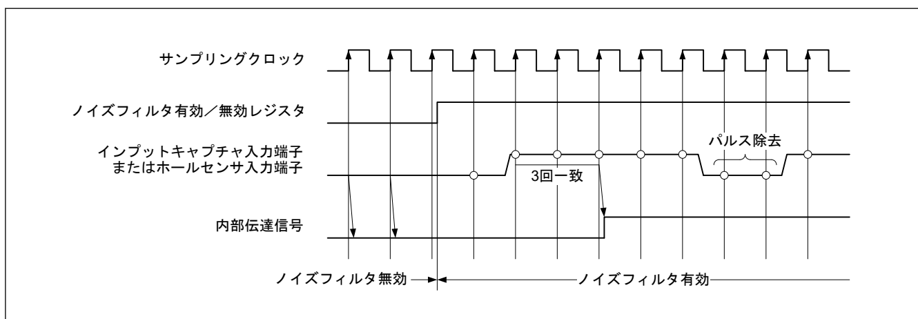
図 21.63 ノイズフィルタのタイミング
