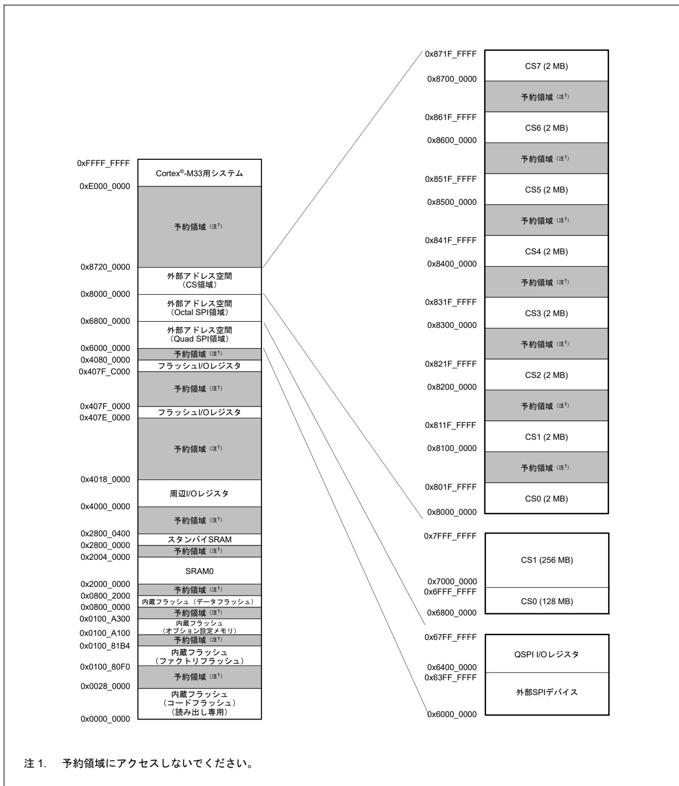
図 4.2 外部アドレス空間と CS 領域の対応関係
