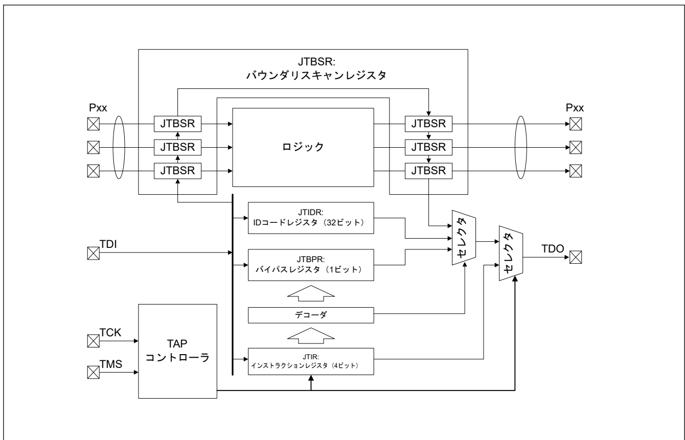
図 38.1 バウンダリスキャン機能のブロック図
