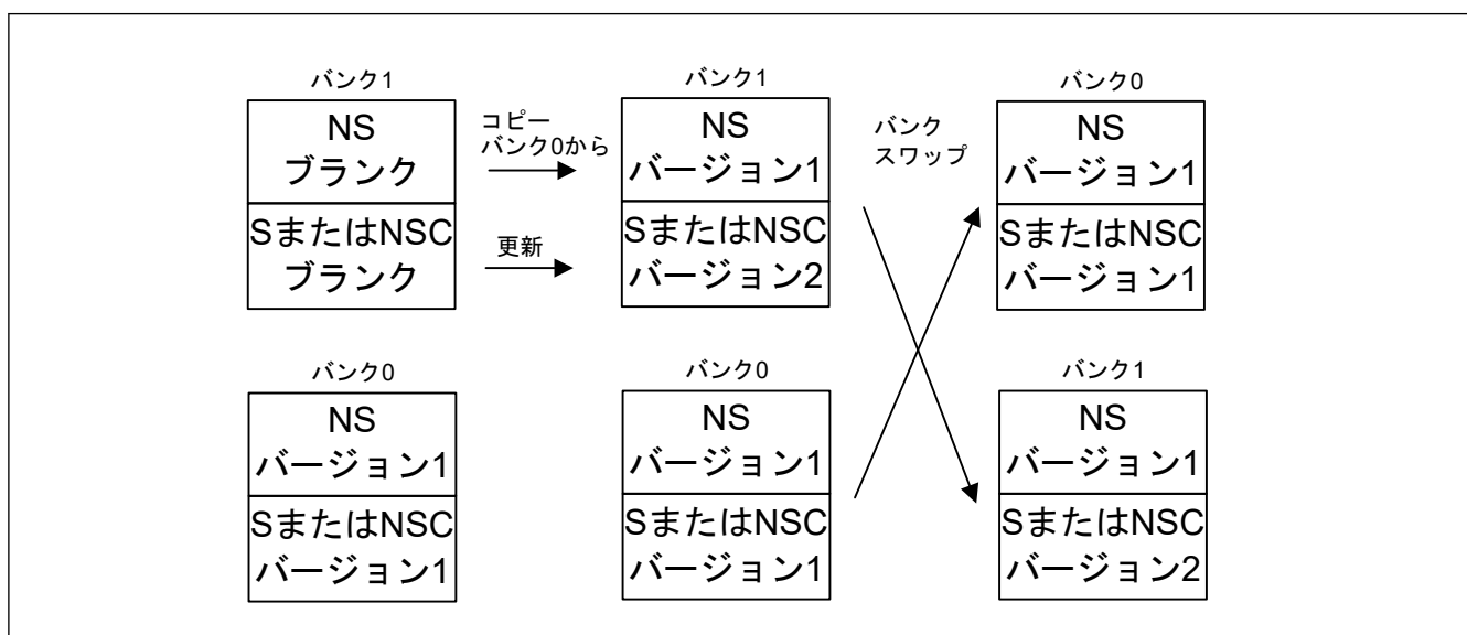
図 49.4 セキュア領域または NSC 領域のフィールドアップデートフロー
