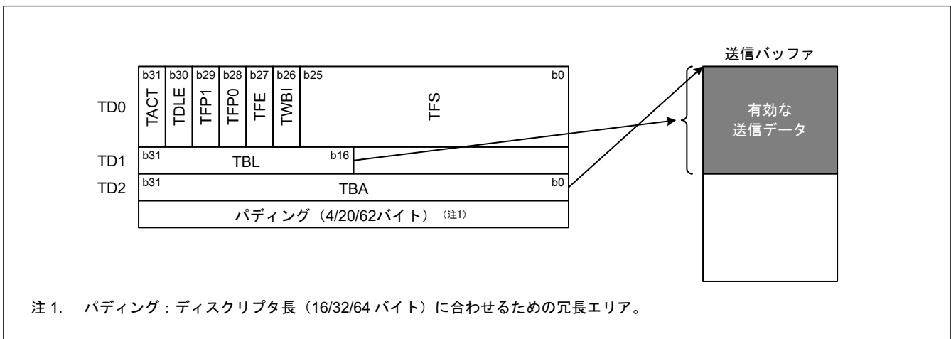
図 27.3 送信ディスクリプタと送信バッファの関係
