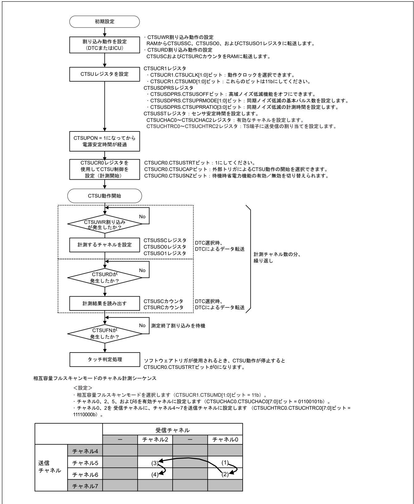
図 43.16 相互容量フルスキャンモードのソフトウェアフローと動作例
