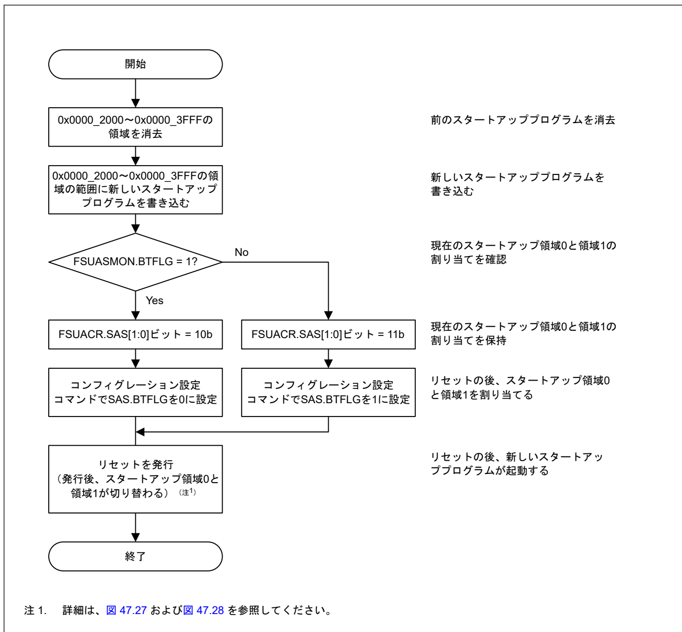
図 47.29 スタートアッププログラムプロテクションの概念
