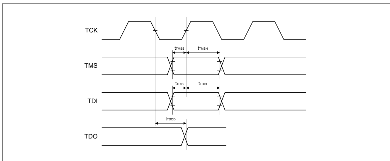
図 50.88 バウンダリスキャン入出カタイミング
