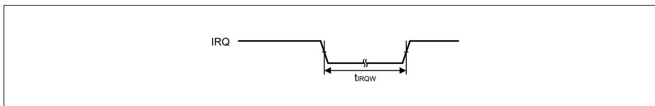
図 50.19 IRQ 割り込み入カタイミング
