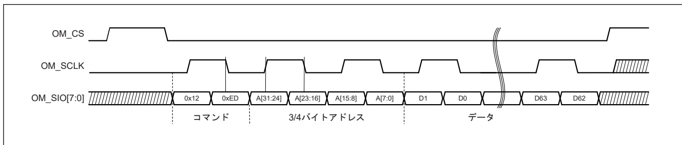
図 34.5 OctaFlash インタフェースでの書き込み動作の波形 (DOPI モード)
