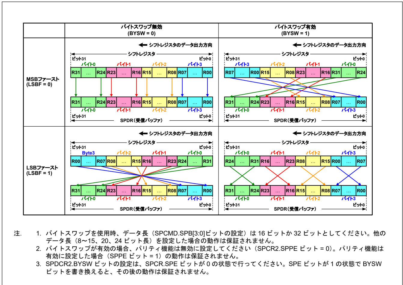
図 32.23 MSB/LSB 転送でのバイトスワップ
