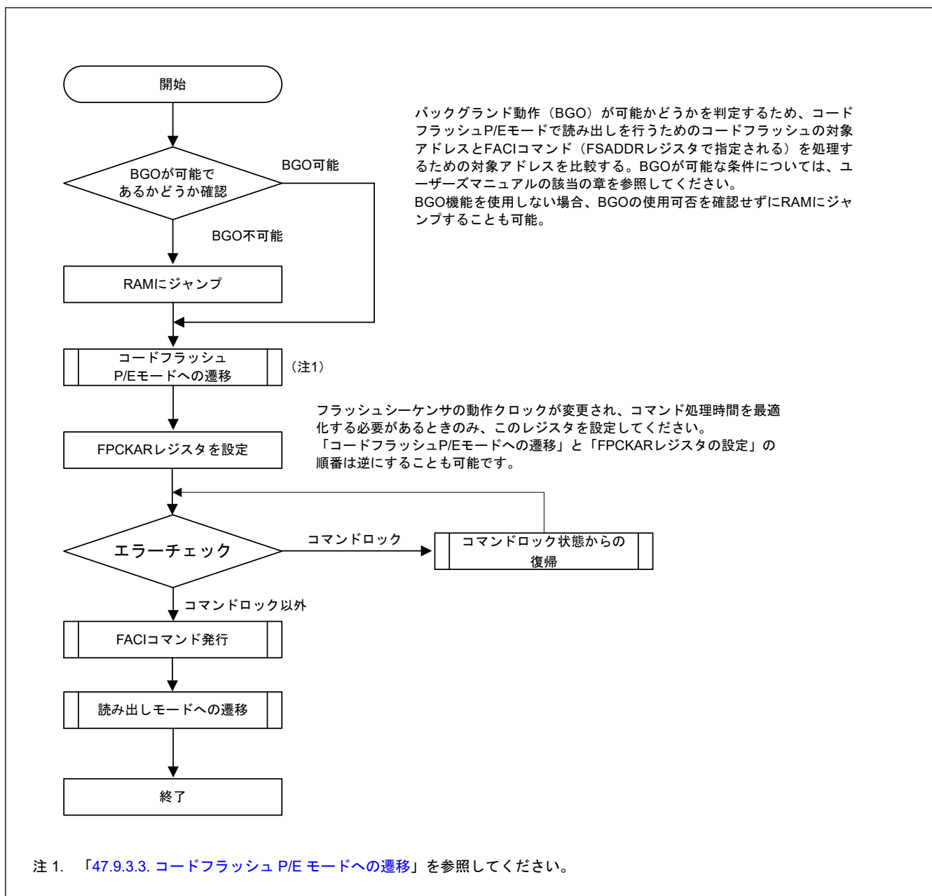
図 47.8 コードフラッシュ P/E モードでのコマンド使用概要
