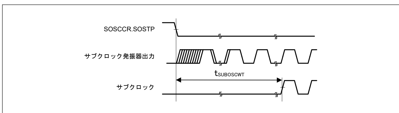
図 50.12 サブクロック発振開始タイミング
