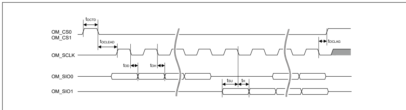
図 50.52 SPI 転送フォーマット送受信タイミング
