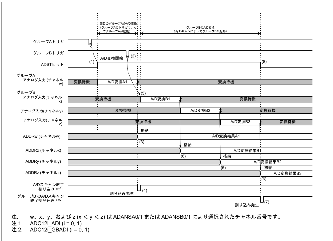
図 40.21 グループ優先動作の例 1-3 : グループ A スキャン中のグループ B トリガ入力、再スキャンあり (ADGSPCR.GBRSCN = 1、ADGSPCR.GBRP = 0、および ADGSPCR.LGRRS = 0 の場合)
