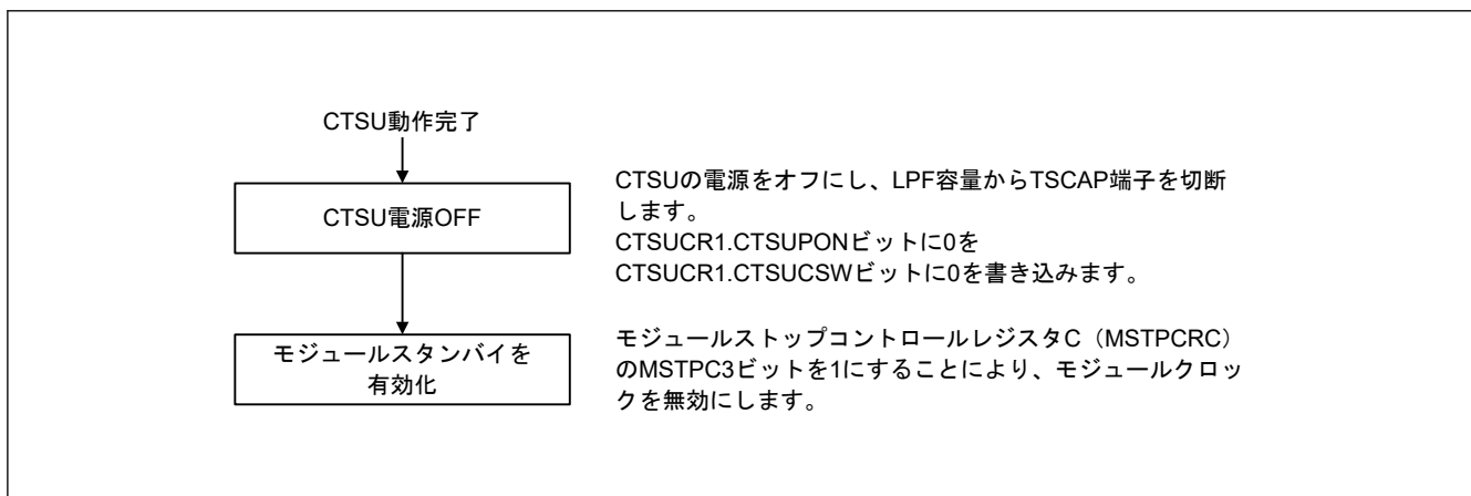
図 43.10 CTSU 停止フロー
