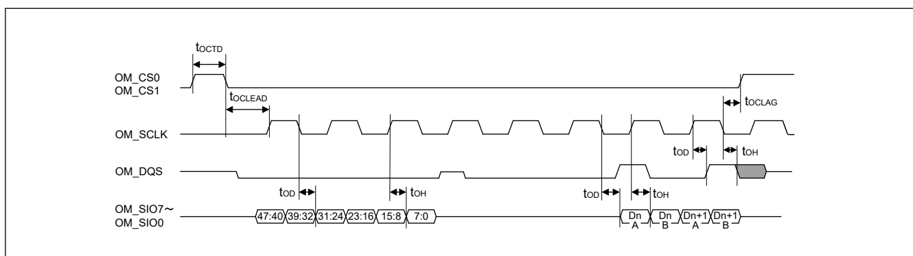
図 50.55 DOPI 転送フォーマット送信タイミング
