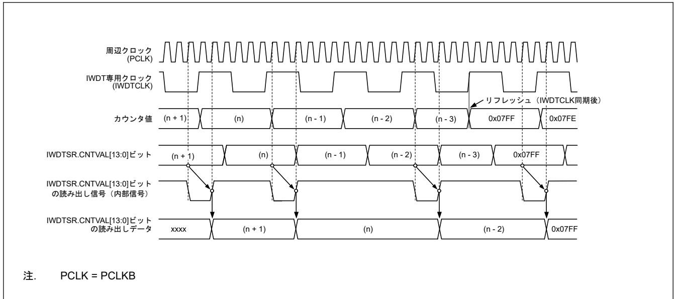
図 25.5 IWDT ダウンカウンタ値の読み出し処理 (OFS0.IWDTCKS[3:0] = 0000b、OFS0.IWDTTOS[1:0] = 11b の場合)
