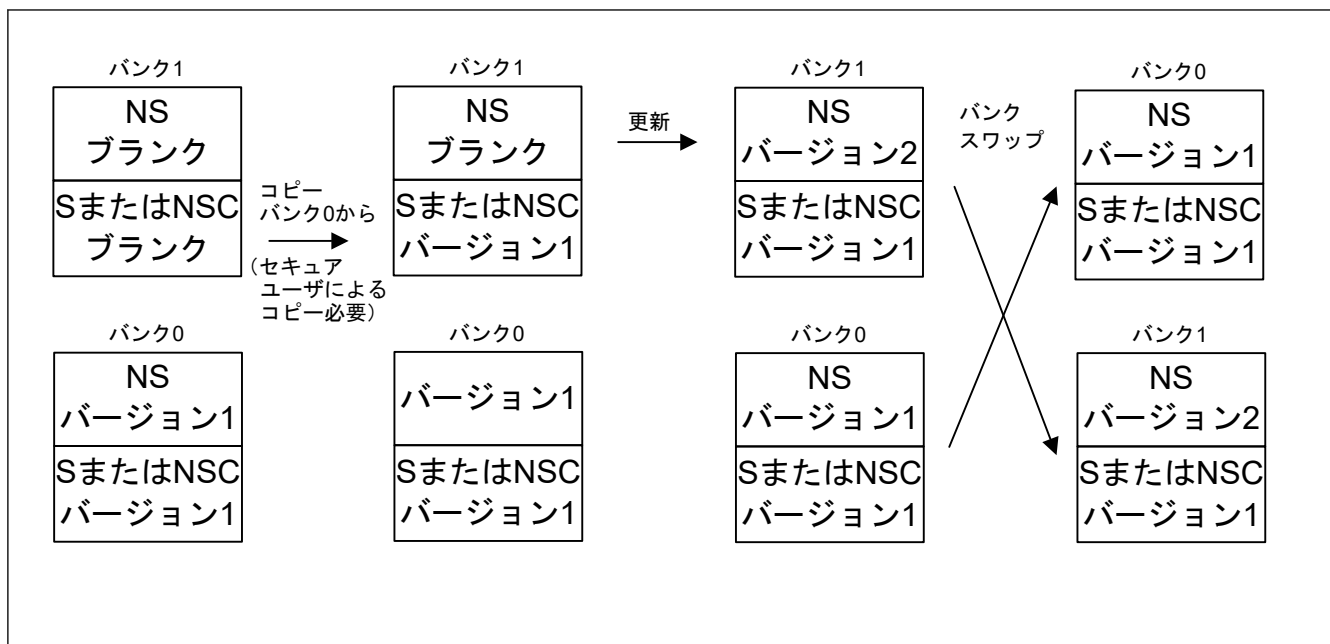
図 49.5 非セキュア領域のフィールドアップデートフロー
