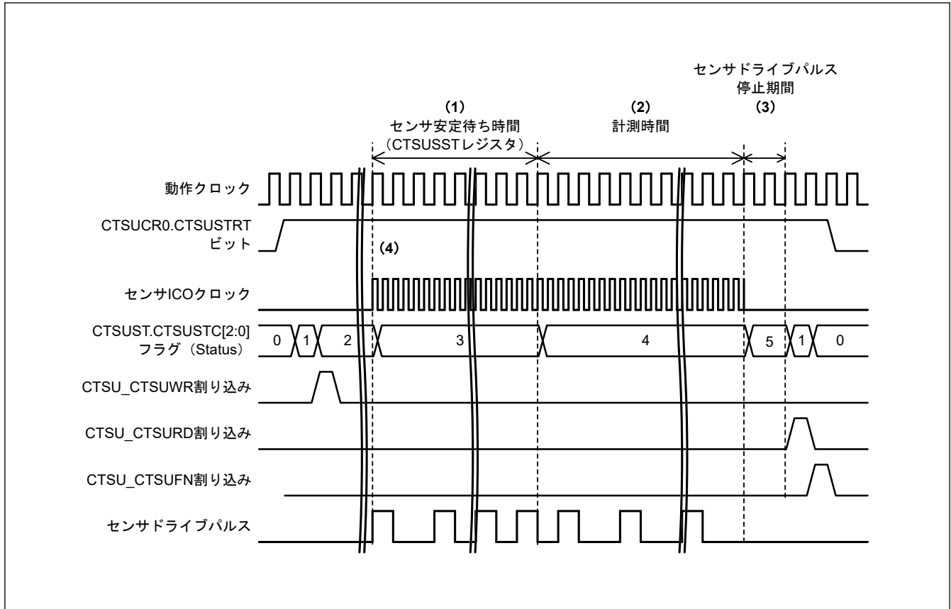
図 43.18 センサ安定待ちと計測のタイミング
