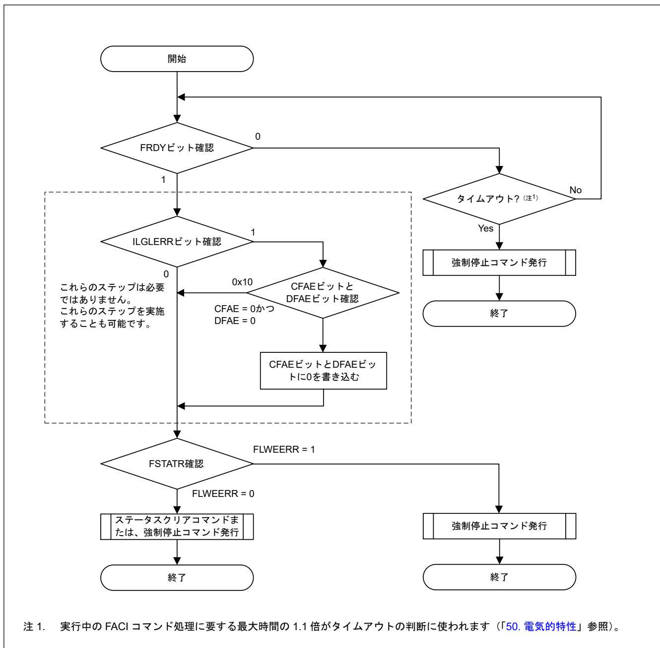
図 47.13 コマンドロック状態からの復帰フロー
