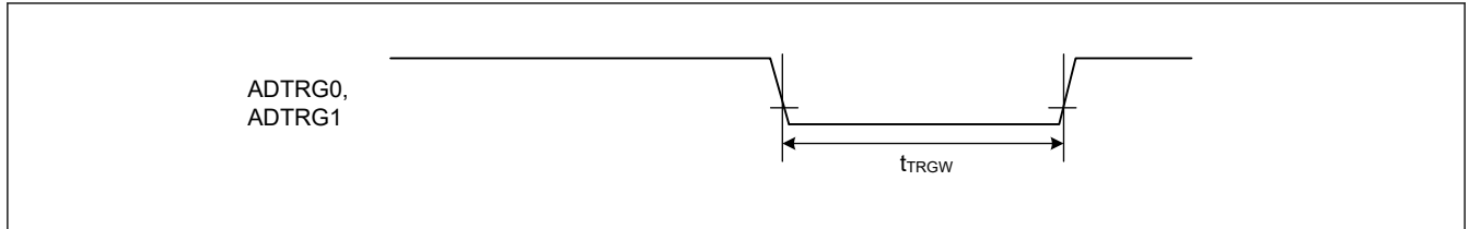
図 50.33 ADC12 トリガ入力タイミング
