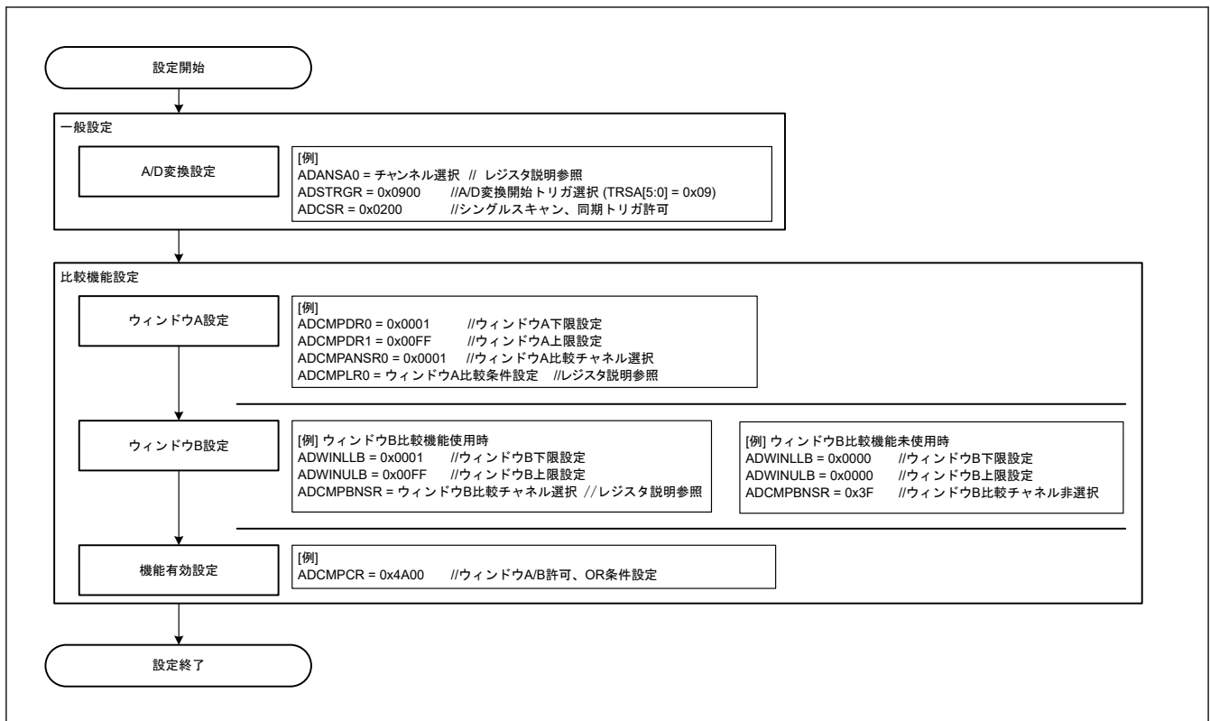
図 40.29 コンペア機能のイベント出力使用時の設定例
