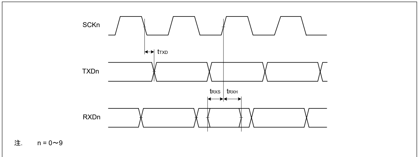
図 50.35 クロック同期式モードにおける SCI 入出力タイミング
