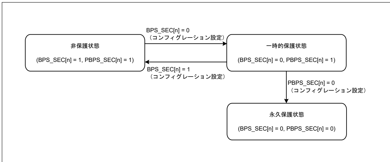
図 47.35 BPS_SEC[n]ビットおよびPBPS_SEC[n]ビットによるフラッシュシーケンサの状態遷移
