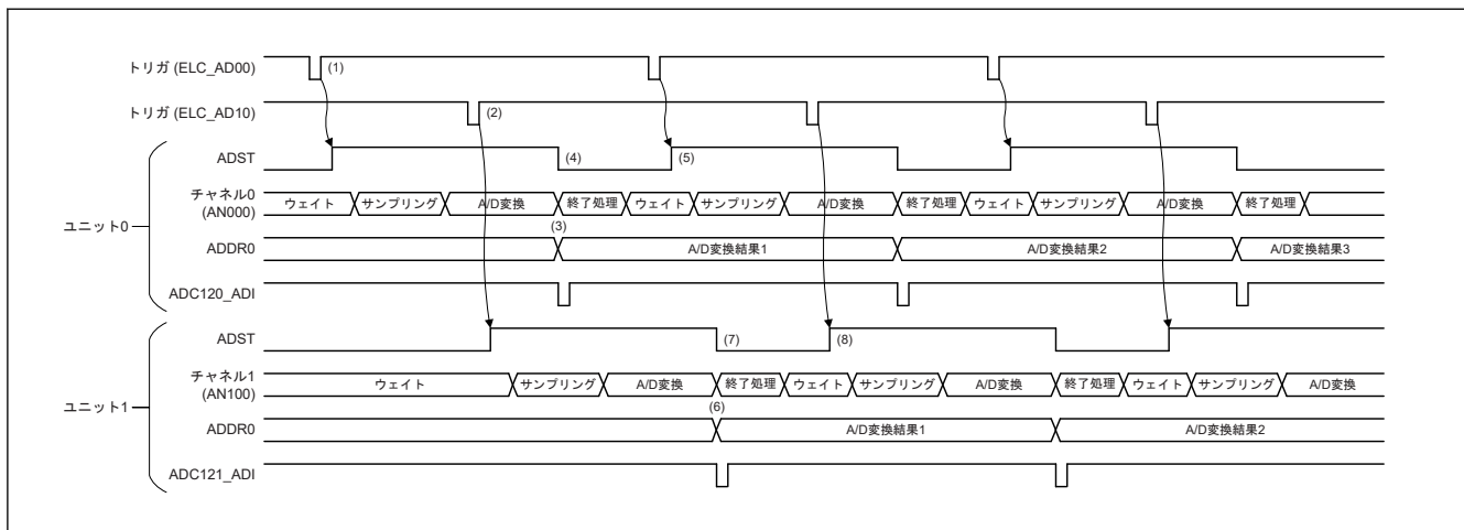
図 40.26 シングルスキャンモードの動作例 (AN000 および AN100 選択、インターリーブ動作)
