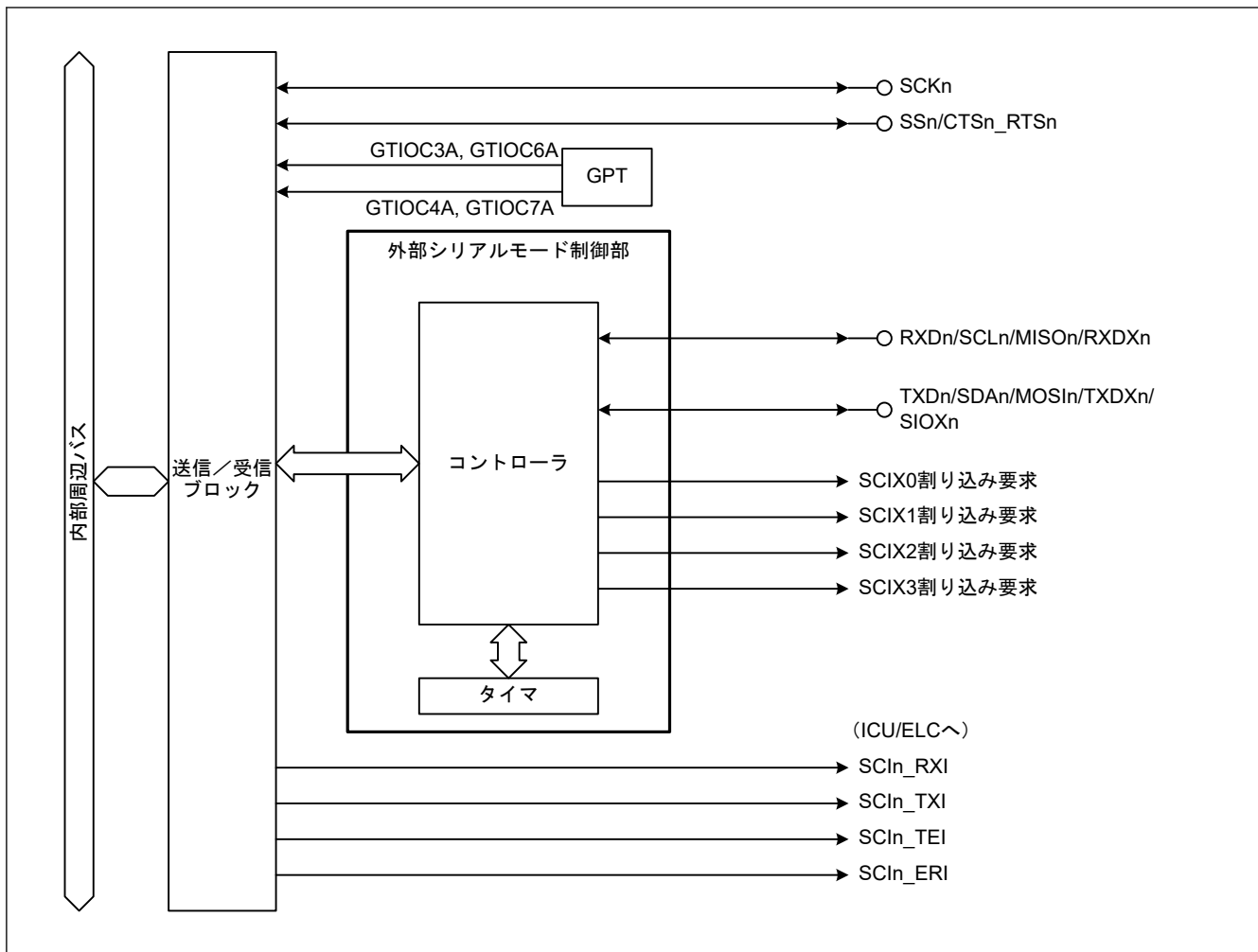
図 29.2 SCI n (n = 1, 2) 拡張シリアルモードコントローラのブロック図
