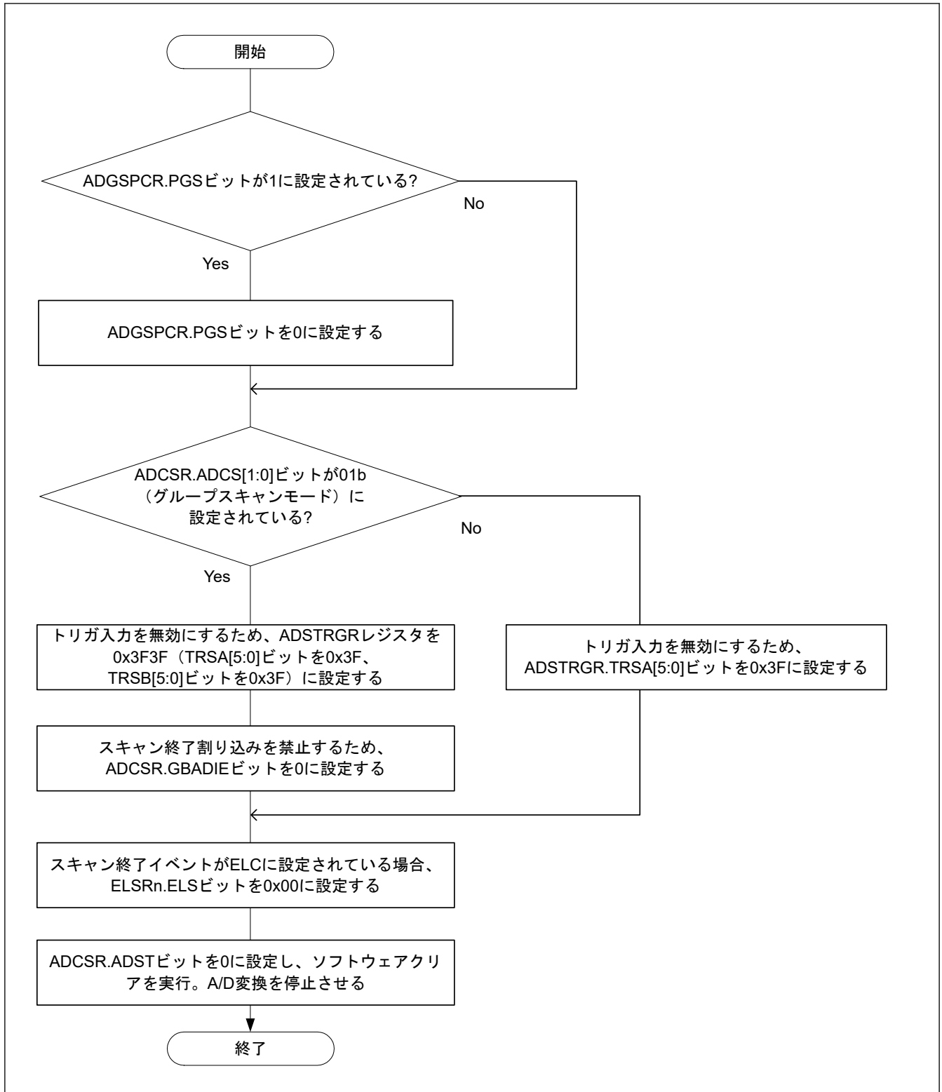
図 40.38 ソフトウェアによる ADCSR.ADST ビットのクリア手順
