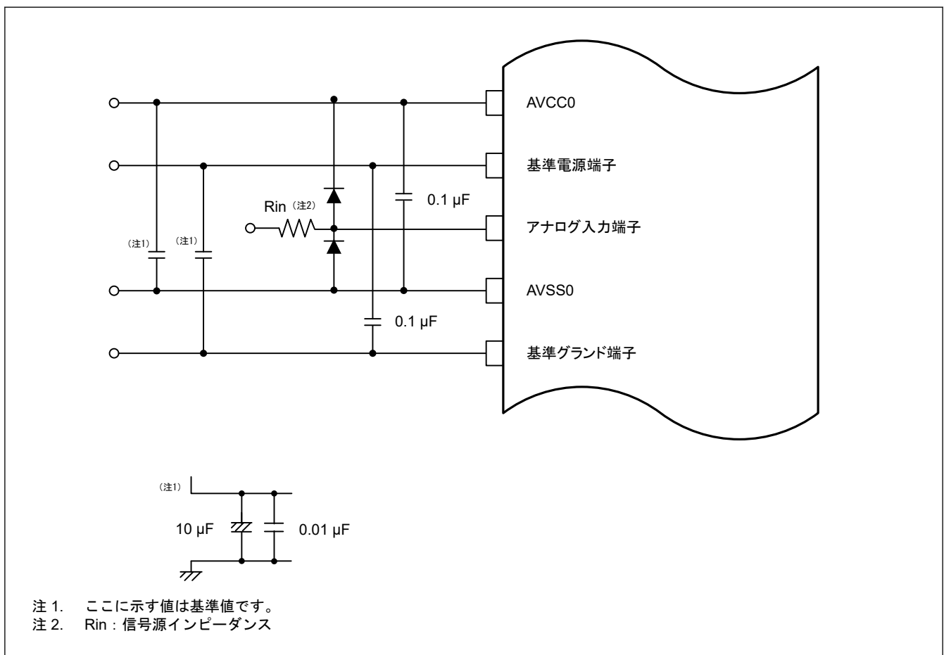
図 40.39 アナログ入力用保護回路例
