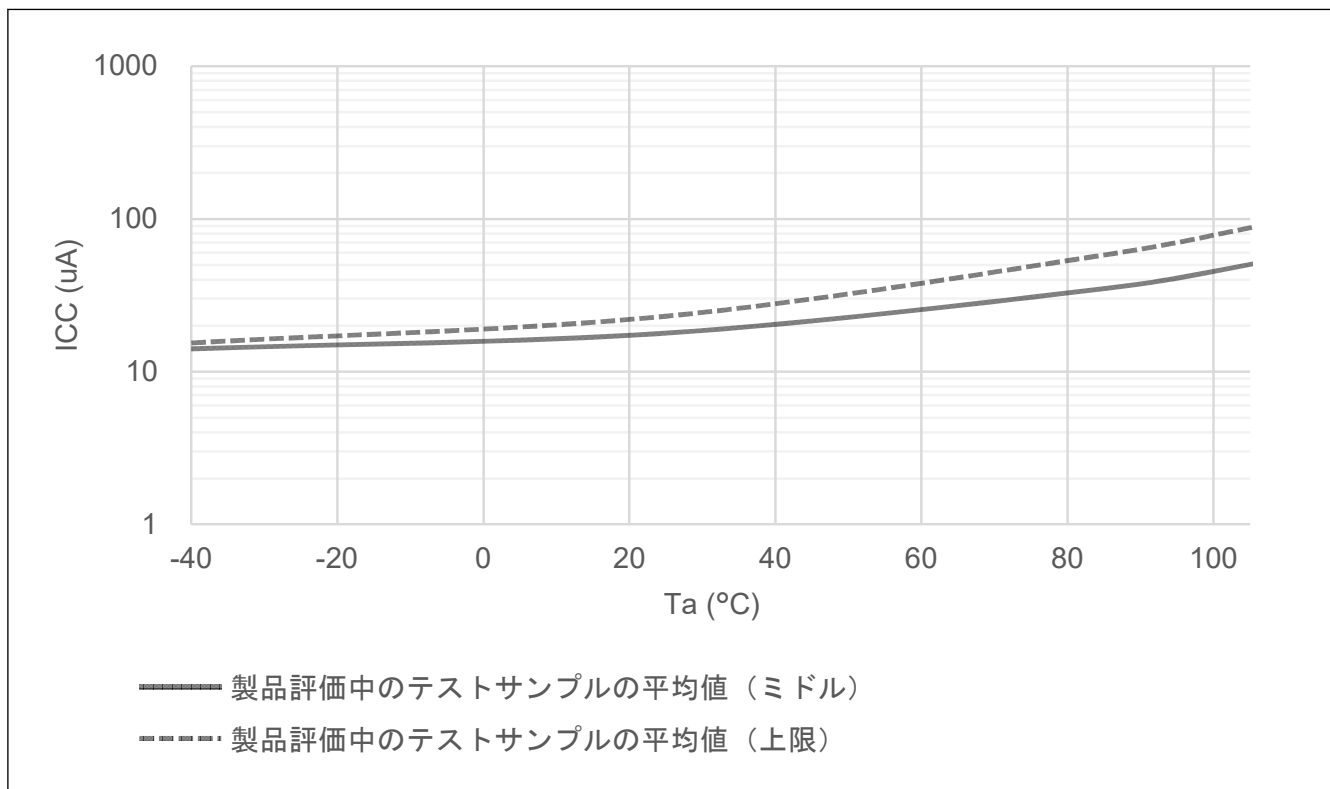
図 50.3 ディープソフトウェアスタンバイモード時の温度依存性、スタンバイ SRAM および USB レジューム検出部への電源供給あり (参考データ)
