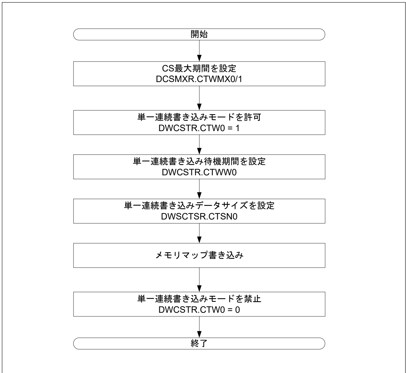
図 34.20 OctaRAM の単一連続書き込み手順
