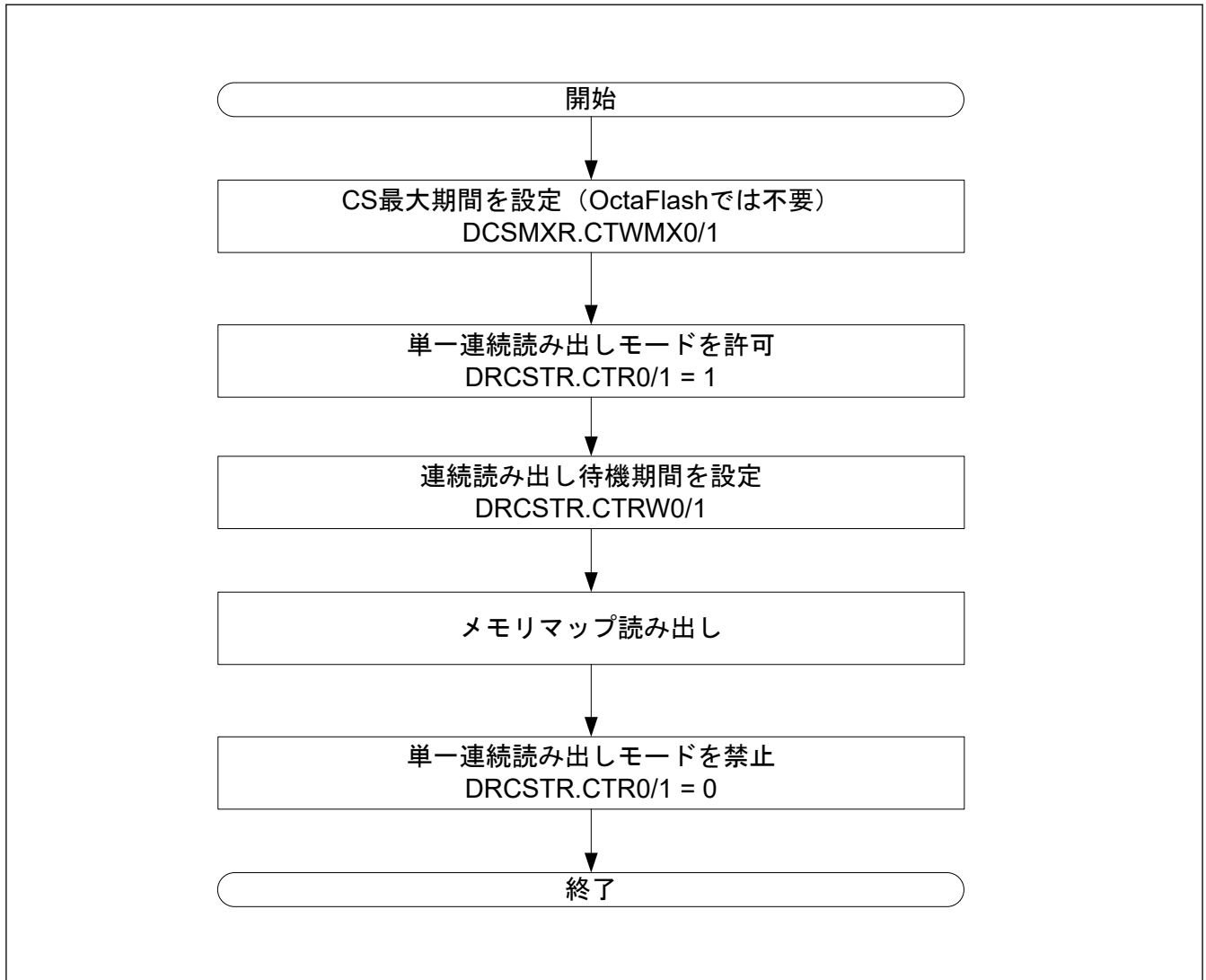
図 34.21 単一連続読み出しの手順
