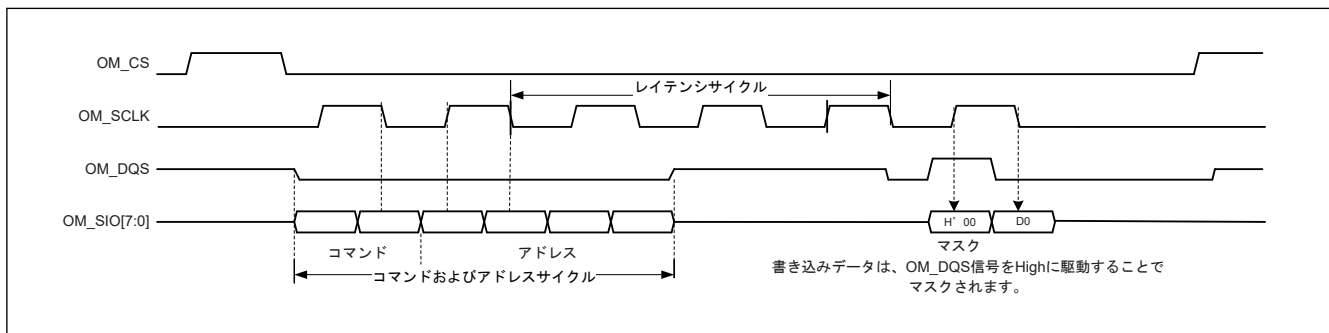
図 34.13 バイトマスクを許可した場合の書き込み動作の波形
