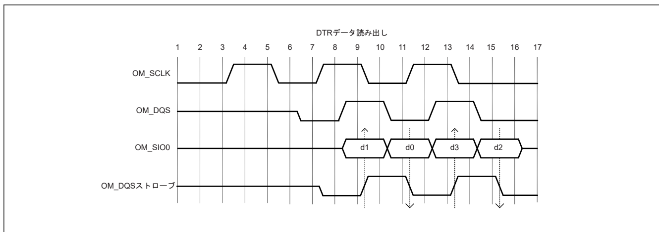
図 34.19 遅延 OM_DQS クロックを使用したデータのラッチ
