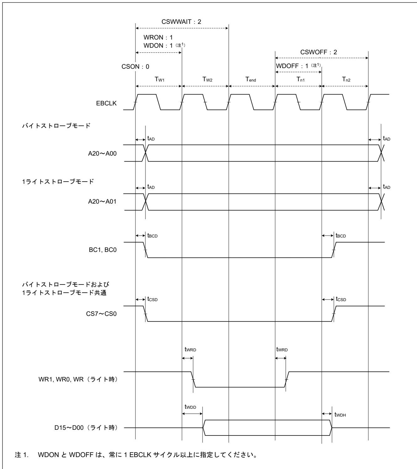
図 50.23 バスクロック同期を使用したノーマルライトサイクルの外部バスタイミング
