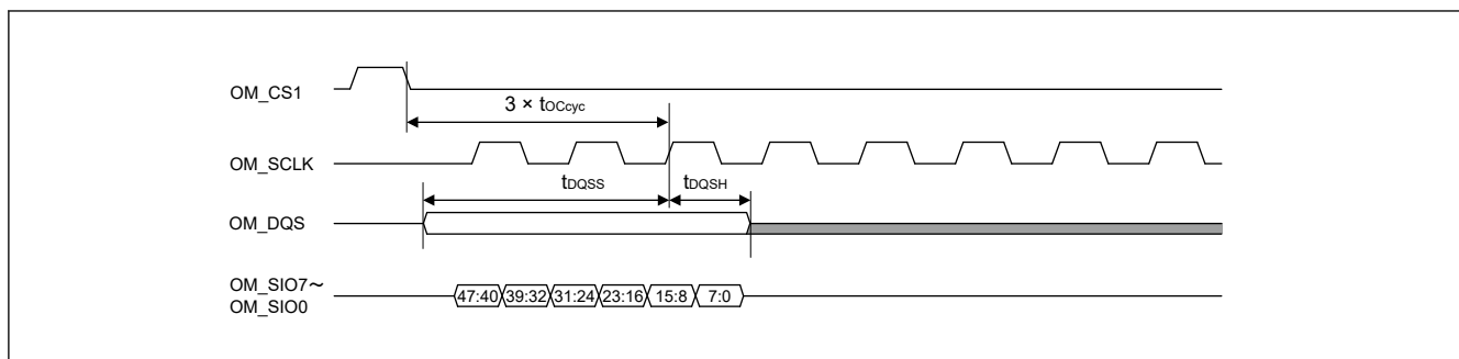
図 50.56 DQS リフレッシュ入力タイミング (OctaRAM™読み出し/書き込み)
