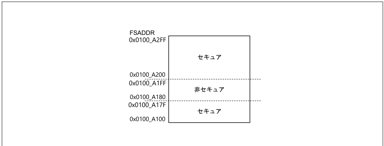
図 47.38 オプション設定メモリのセキュア/非セキュア領域
