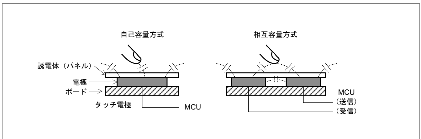
図 43.2 自己容量方式と相互容量方式
