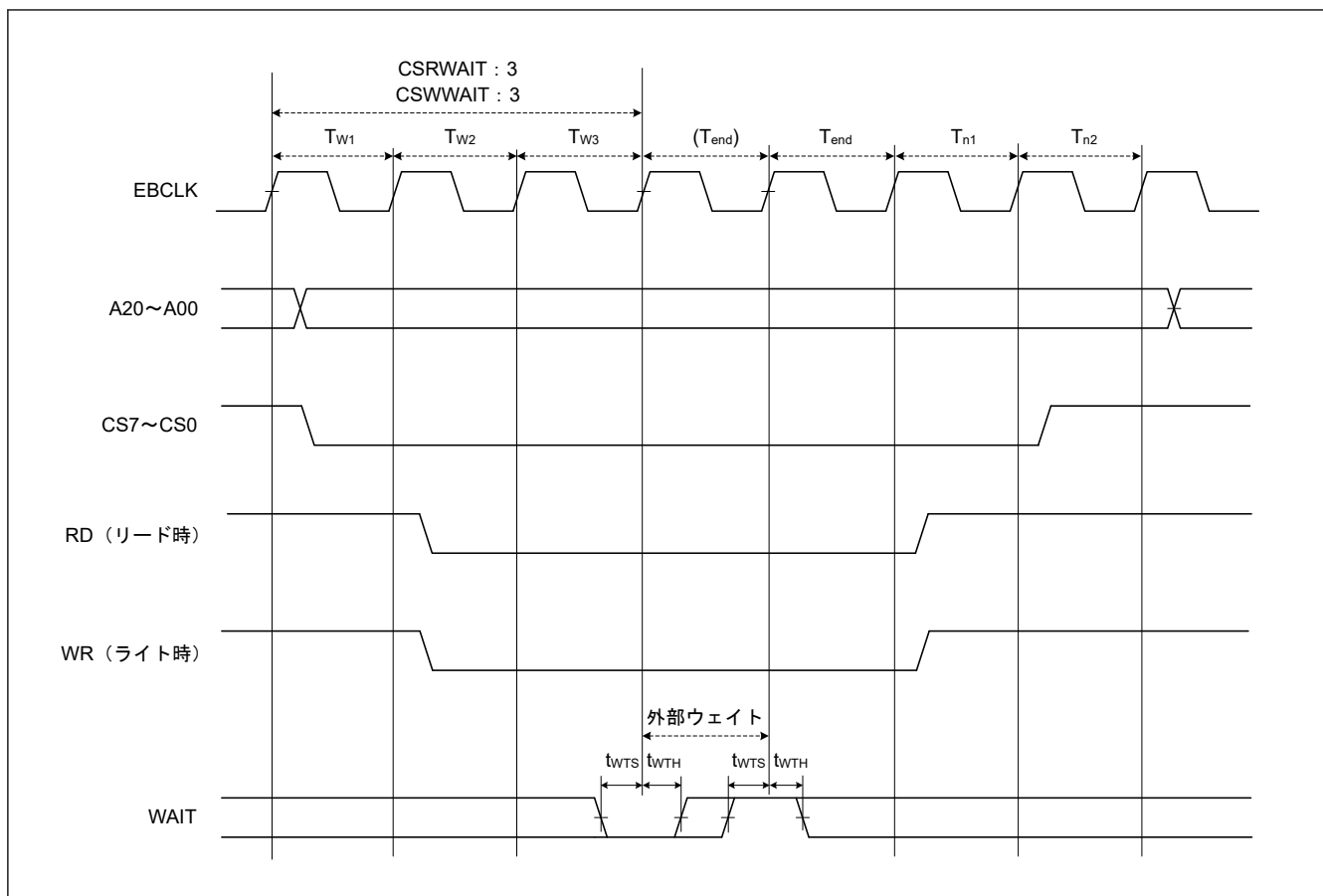
図 50.26 外部ウェイト制御の外部バスタイミング
