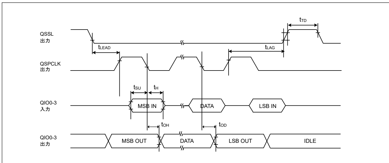
図 50.50 送受信タイミング
