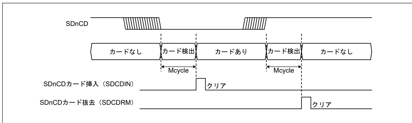
図 36.7 SDnCD によるカード検出例
