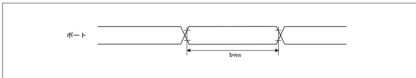
図 50.27 I/O ポート入力タイミング
