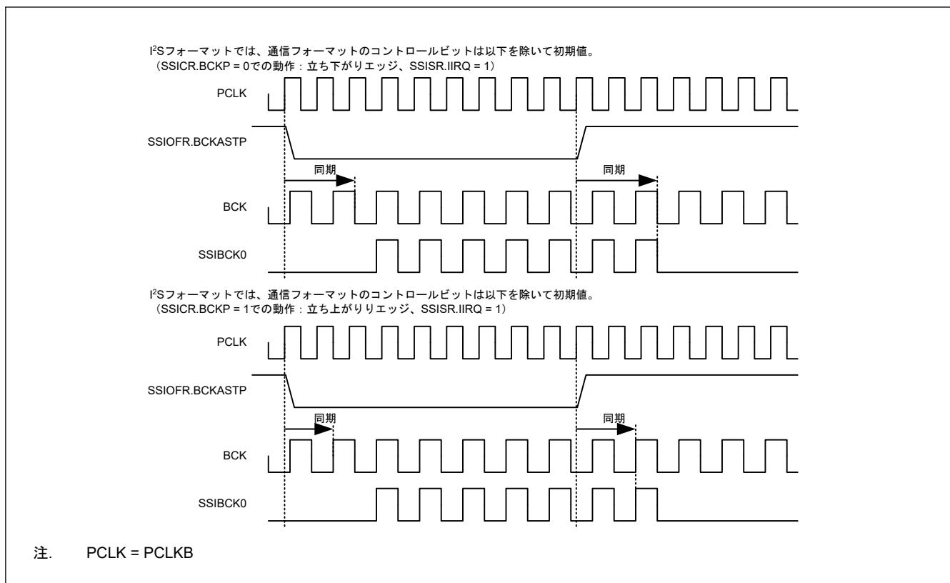
図 35.45 SSIOFR.BCKASTP による SSIBCK0 停止の例
