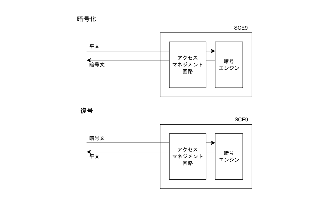
図 39.2 暗号エンジンの概念図
