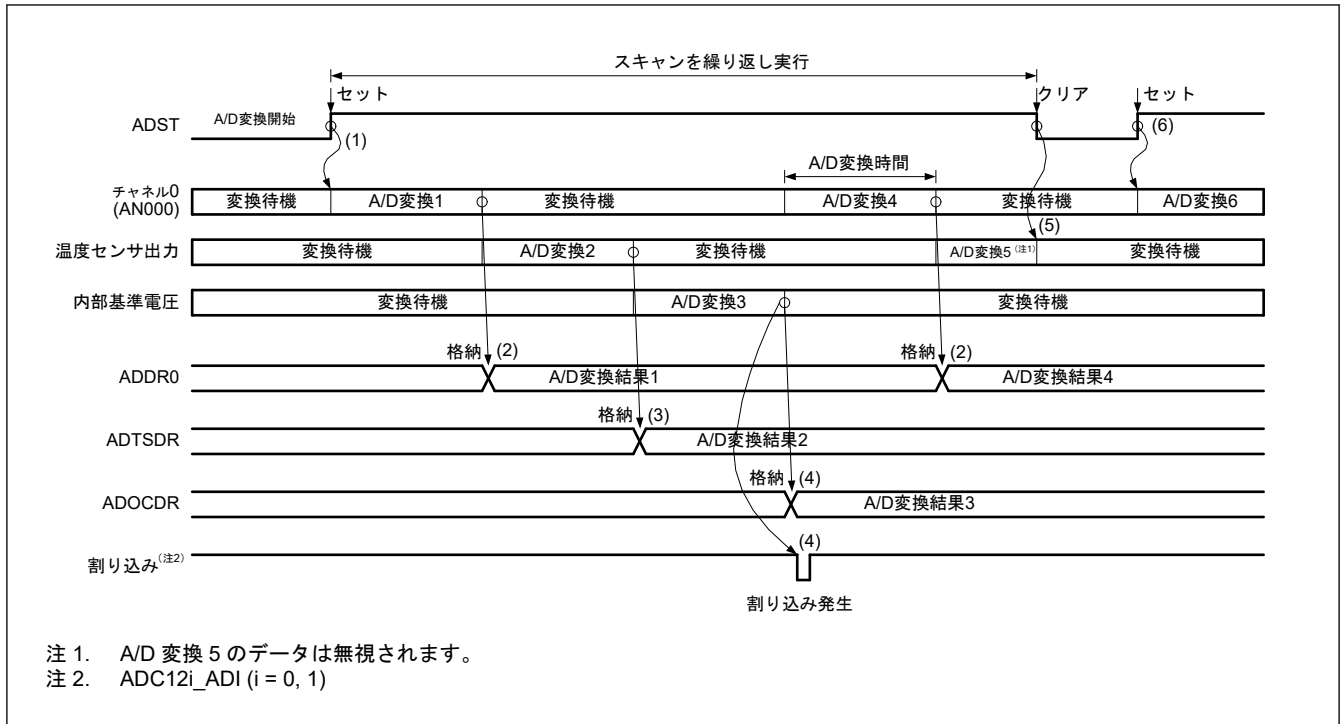
図 40.15 連続スキャンモードの基本動作例 (AN000、温度センサ出力または内部基準電圧選択)
