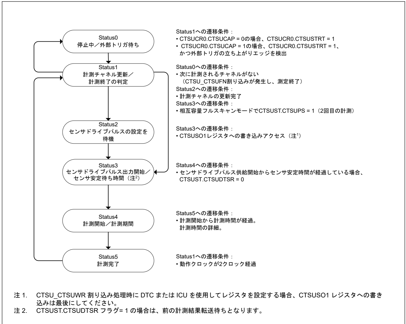
図 43.11 ステータス動作遷移図
