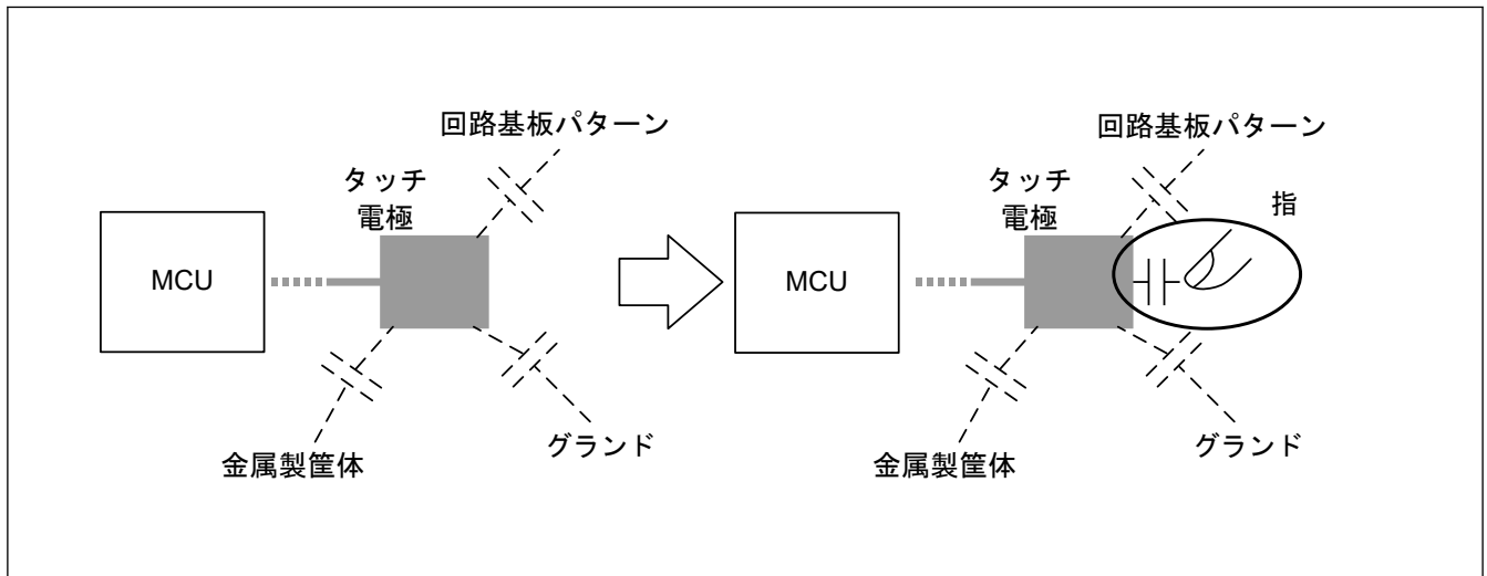
図 43.1 指による静電容量の増加
