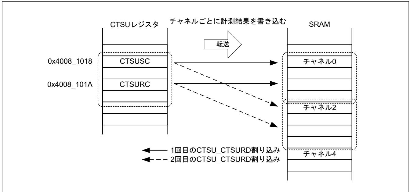
図 43.20 CTSU_CTSURD 割り込みを用いた DTC 転送動作例
