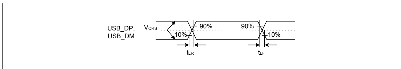
図 50.74 Low-speed モードにおける USB_DP、USB_DM の出力タイミング
