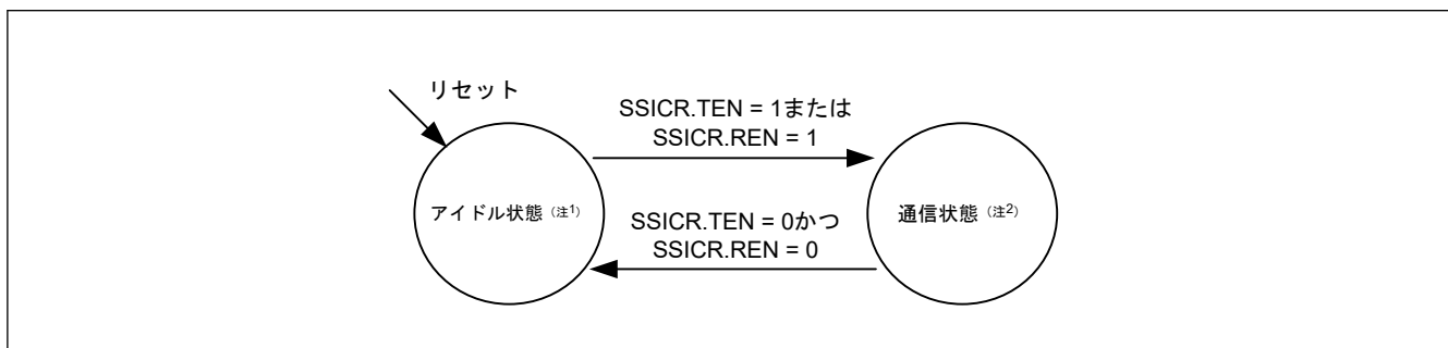
図 35.43 SSIE の状態遷移
