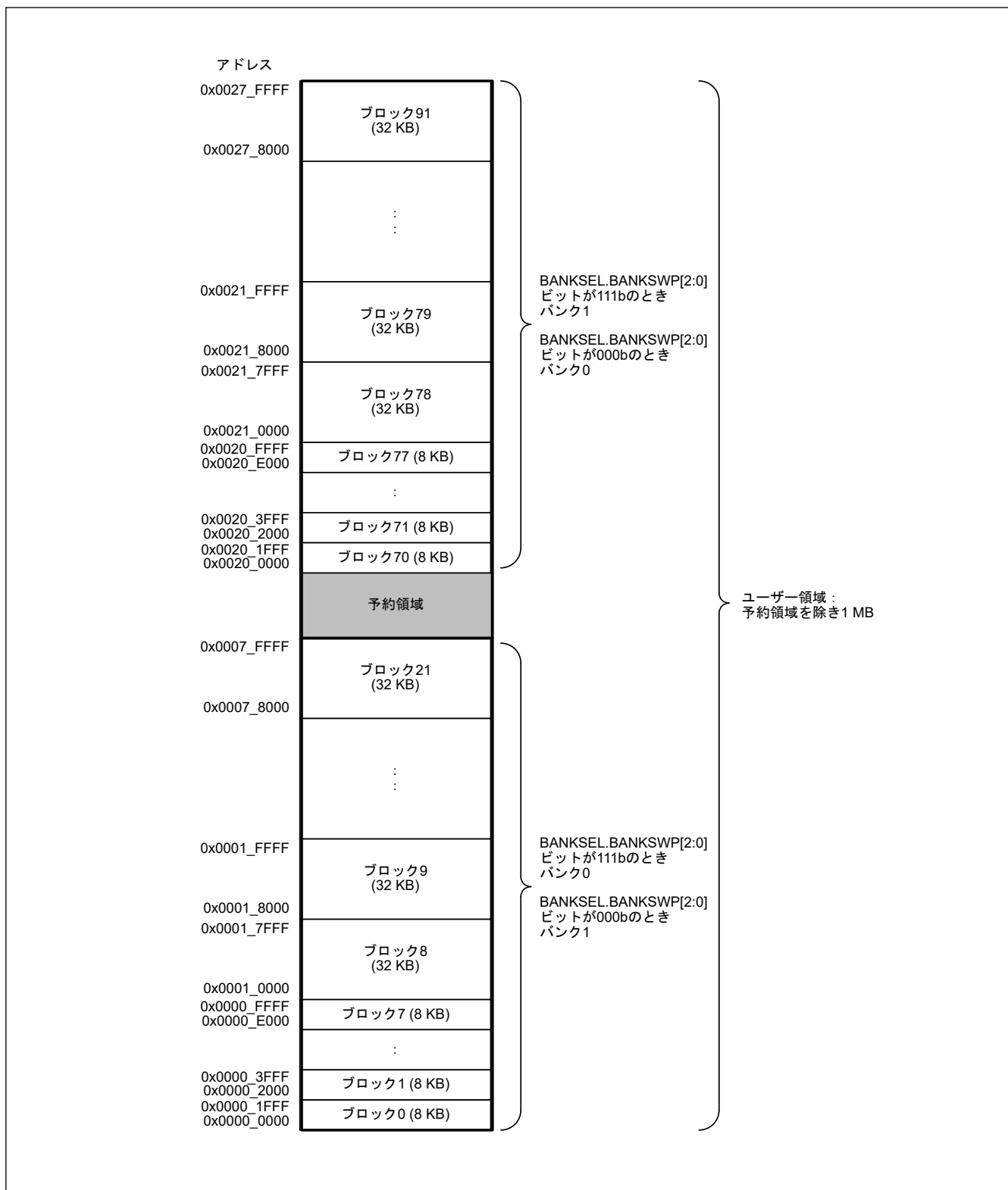
図 47.3 デュアルモードでのコードフラッシュメモリのマップ
