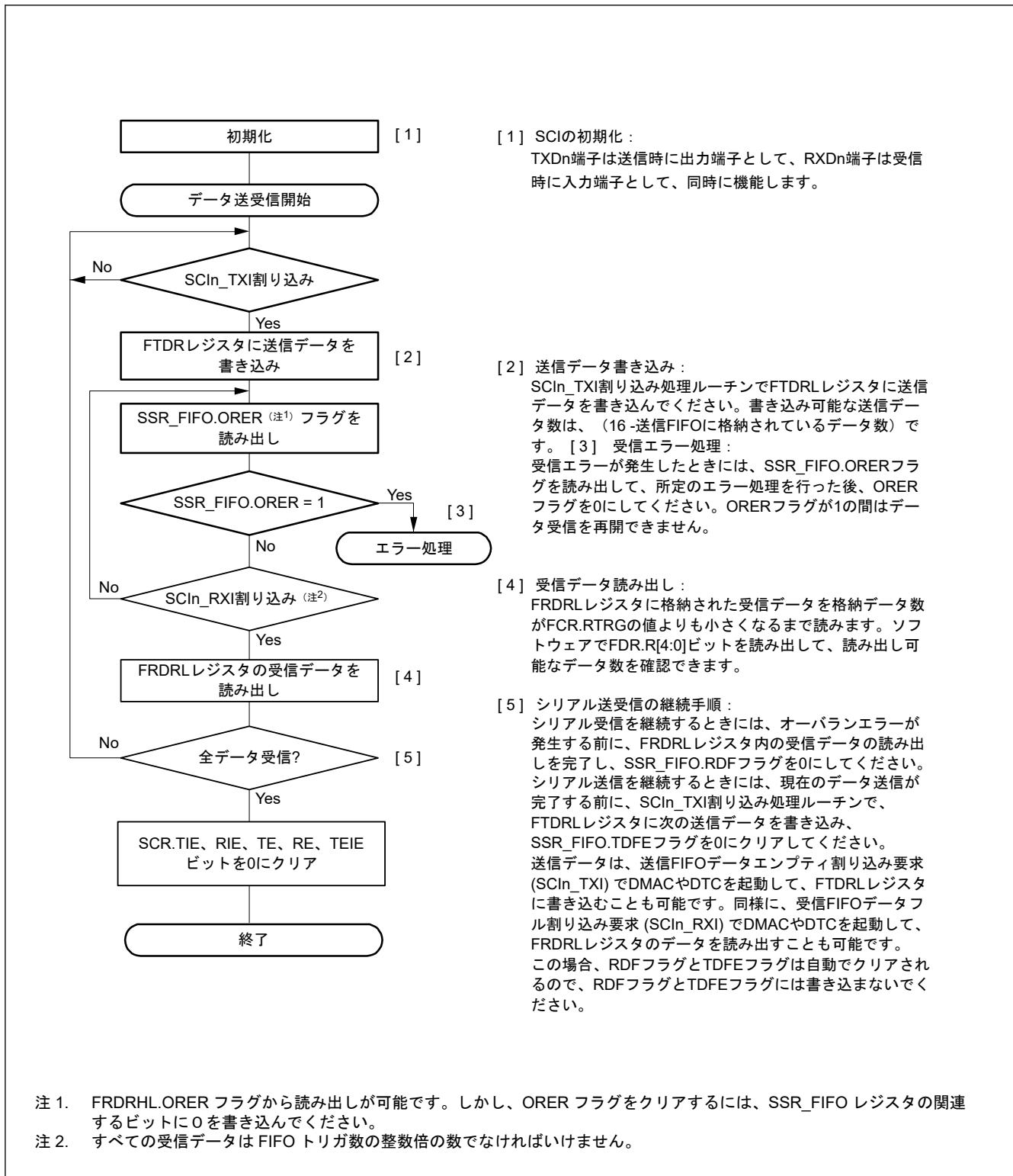
図 29.76 クロック同期式モードにおけるシリアル同時送受信動作のフローチャート例 (FIFO 選択時)
