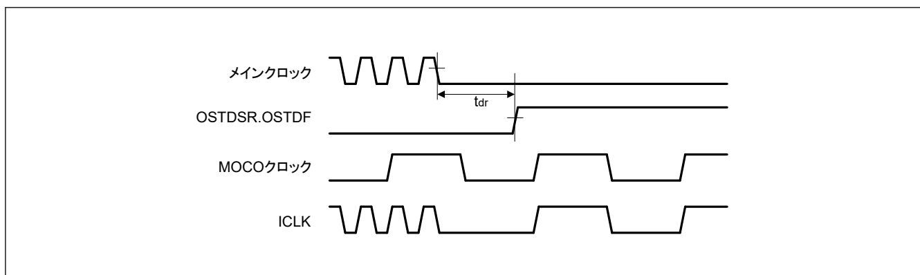
図 50.79 発振停止検出タイミング
