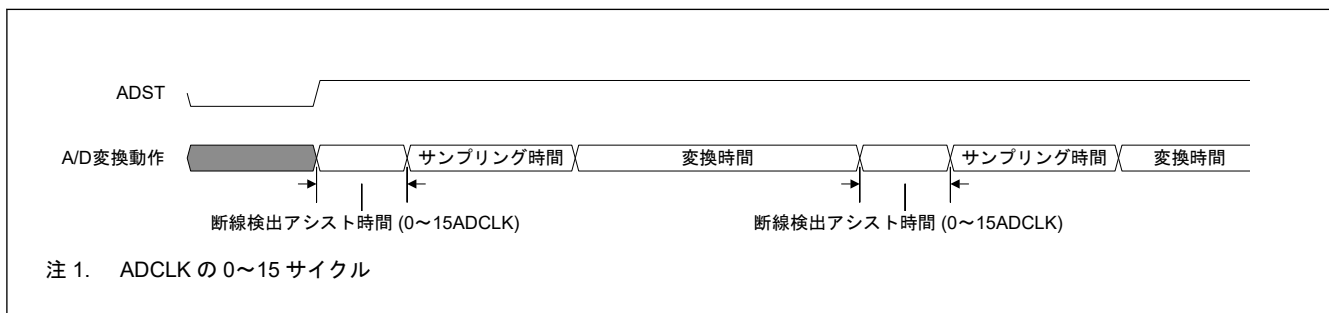
図 40.33 断線検出アシスト機能を使用した場合の A/D 変換動作図
