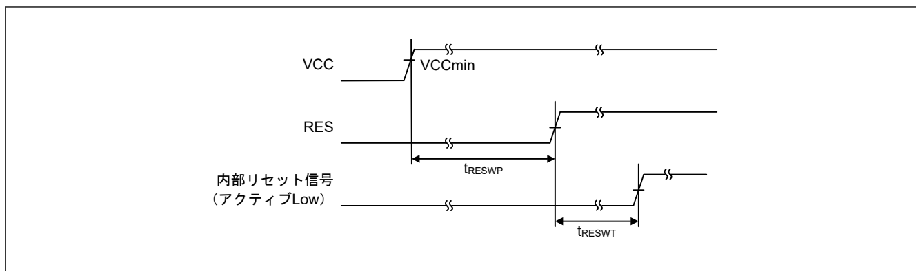
図 50.13 VCC が V POR 電圧しきい値を超える条件下での RES 端子入力タイミング
