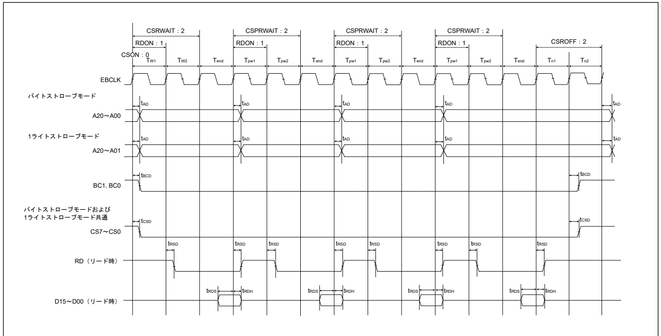
図 50.24 バスクロック同期を使用したページリードサイクルの外部バスタイミング
