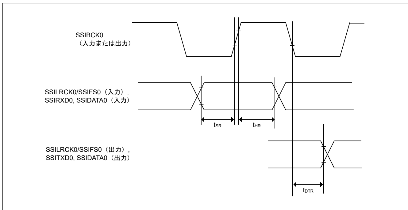
図 50.60 SSICR.BCKP = 0 の場合の SSIE データ送受信タイミング
