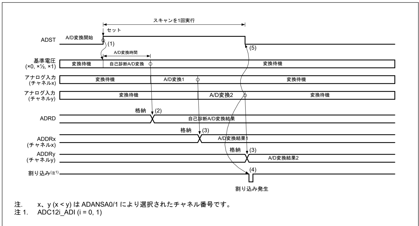
図 40.9 シングルスキャンモードの基本動作例 (アナログ入力 (チャンネル x、y) 選択+自己診断)
