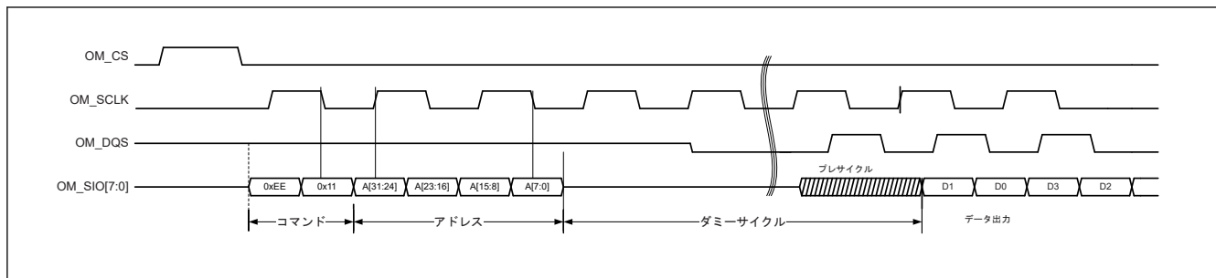
図 34.9 OctaFlash インタフェースでの読み出し動作の波形 (プレサイクル許可を使用した DOPI モード)
