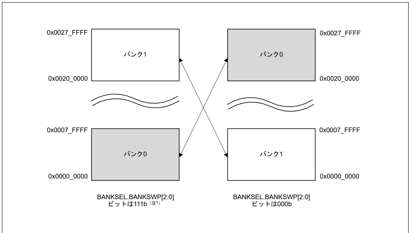
図 47.31 スタートアップバンク選択例 (1 M バイトのコードフラッシュメモリを持つ製品の場合)
