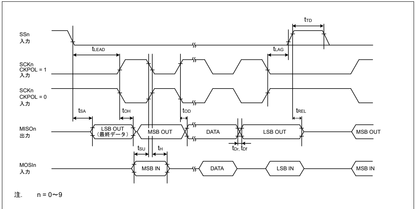
図 50.40 CKPH = 0 の場合におけるスレーブの SCI 簡易 SPI モードタイミング
