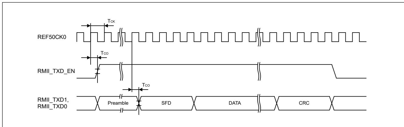
図 50.65 RMIi 送信タイミング
