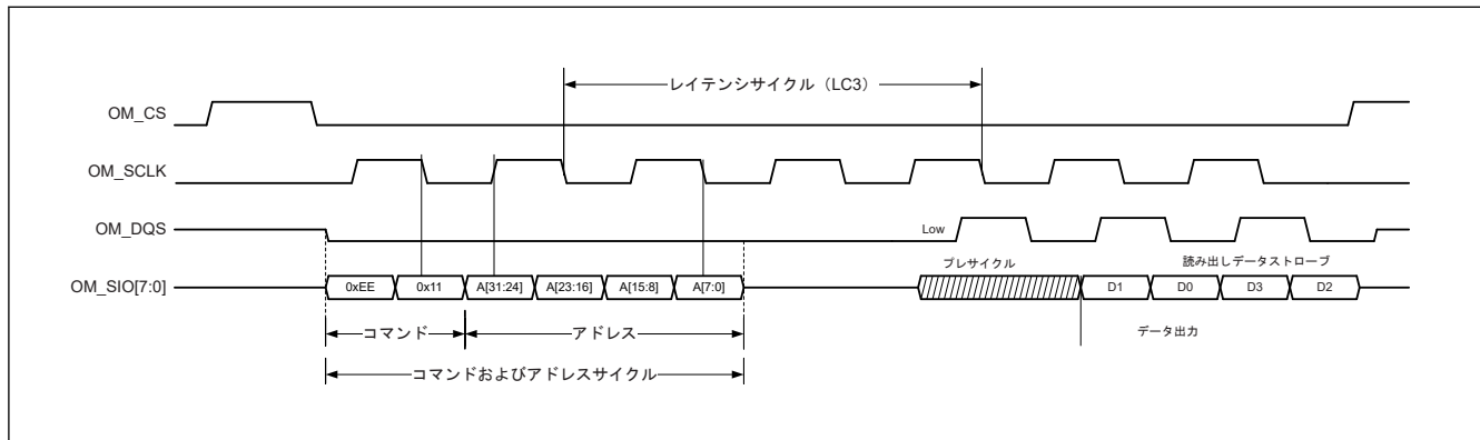
図 34.10 OctaRAM インタフェースでの読み出し動作の波形 (プレサイクル許可を使用した DOPI モード)
