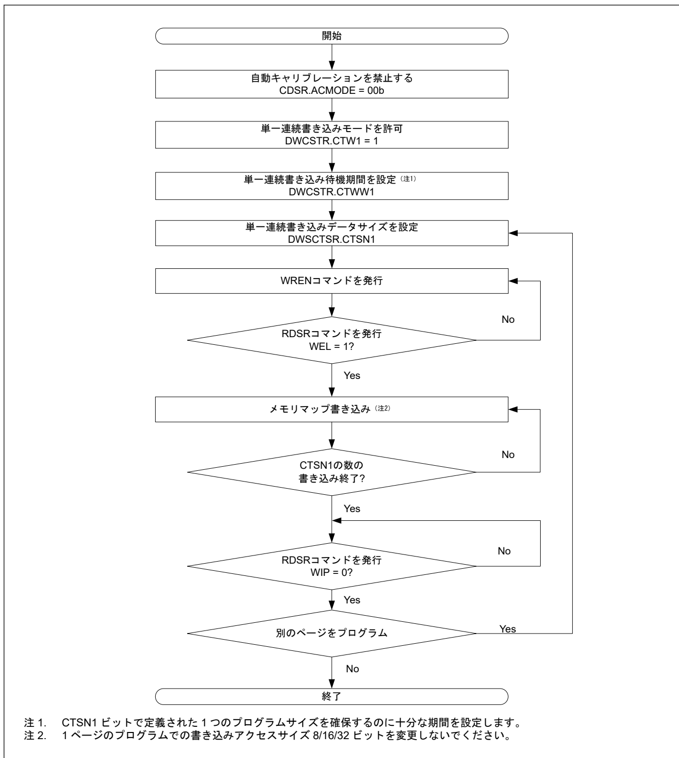
図 34.17 OctaFlash プログラムの手順
