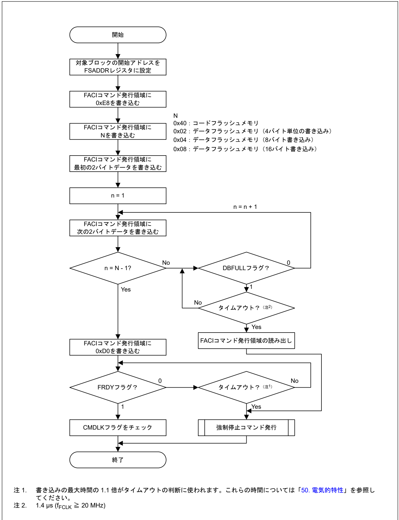
図 47.14 プログラムコマンドの使用フロー
