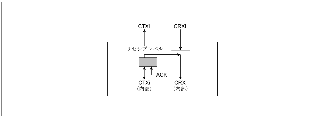
図 31.8 セルフテストモード 1 選択時の接続 ( i = 0, 1 )
