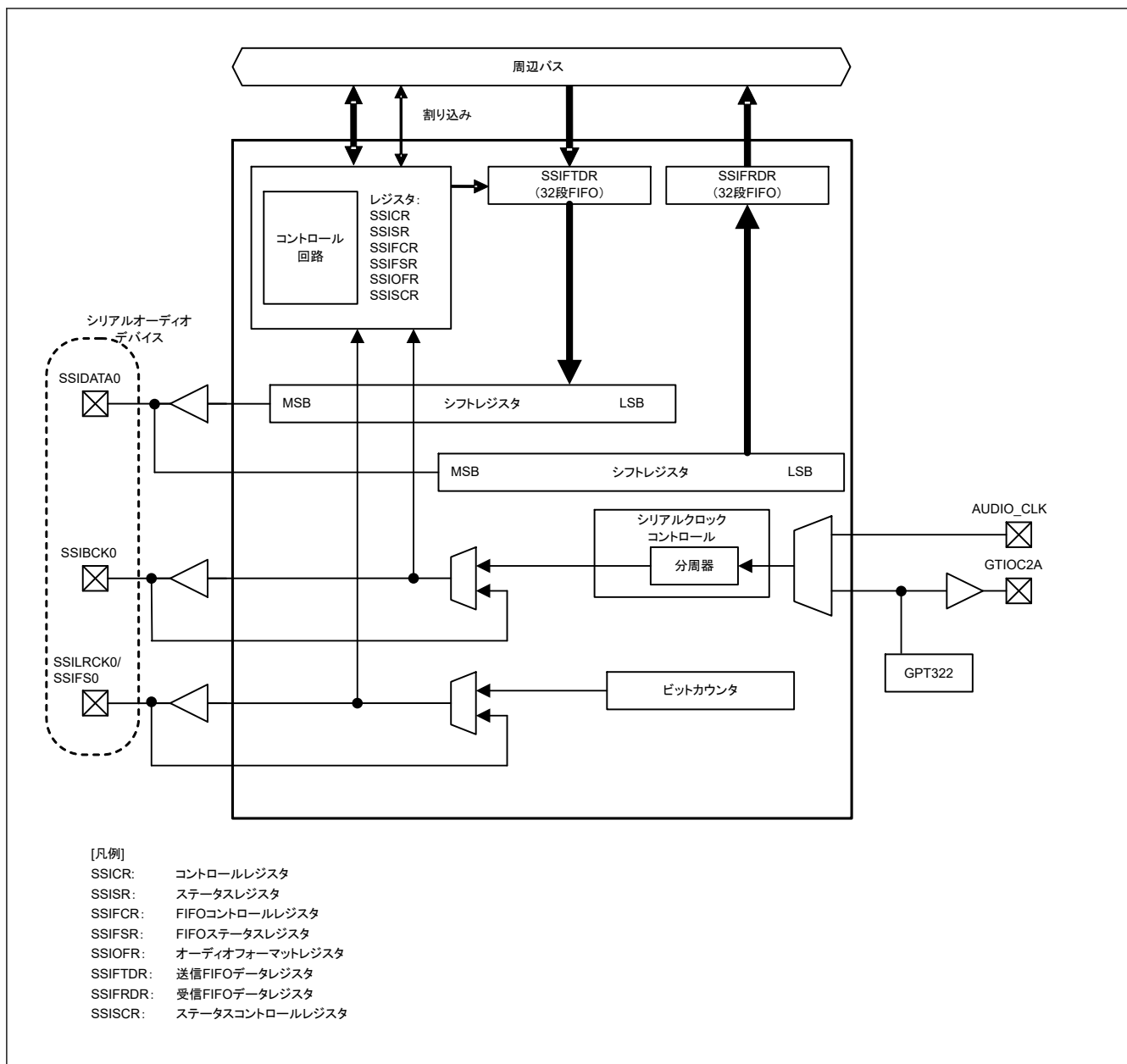
図 35.3 半二重通信の SSIE ブロック図
