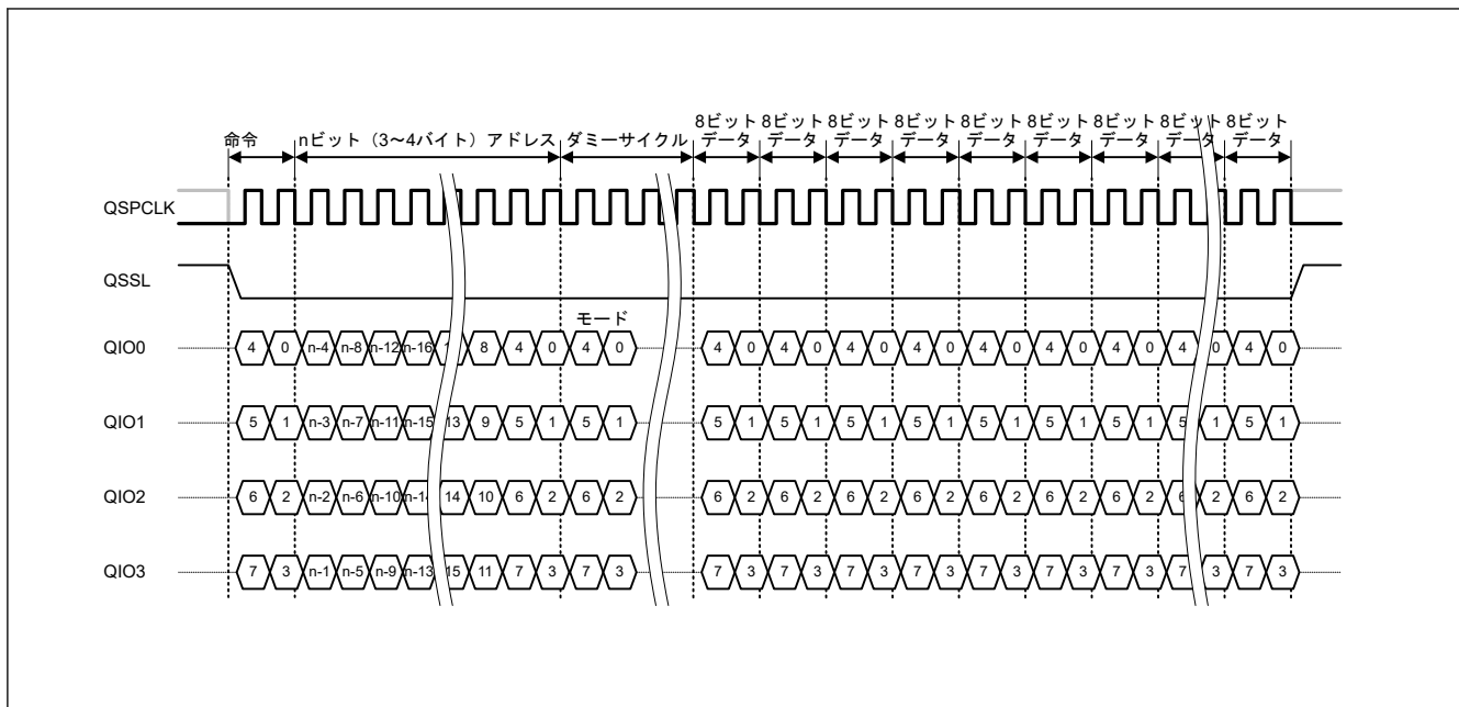
図 33.7 Quad-SPI プロトコル例 (ファストリード Quad I/O)
