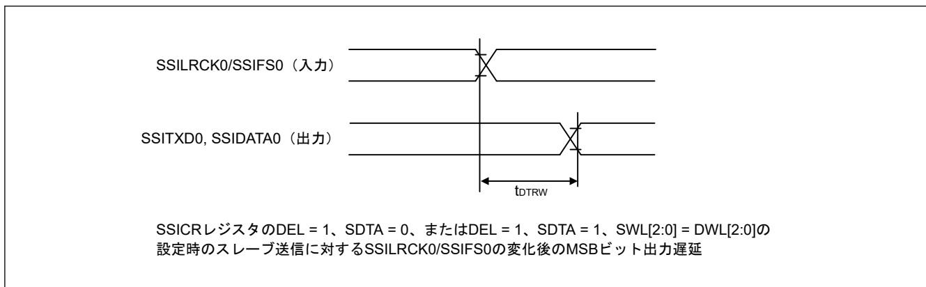
図 50.62 SSILRCK0/SSIFS0 変化時からの SSIE データ出力遅延
