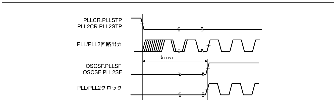
図 50.11 PLL/PLL2 クロック発振開始タイミング
