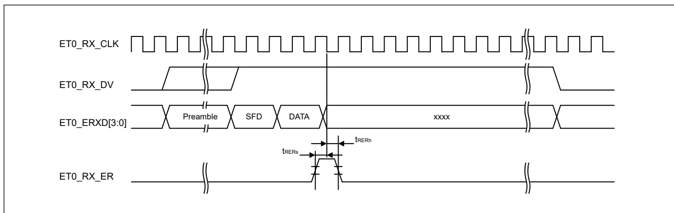
図 50.72 エラー発生時の MII 受信タイミング
