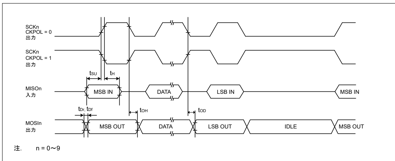
図 50.37 CKPH = 1 の場合におけるマスタの SCI 簡易 SPI モードタイミング
