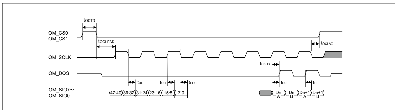
図 50.54 DOPI 転送フォーマット送受信タイミング
