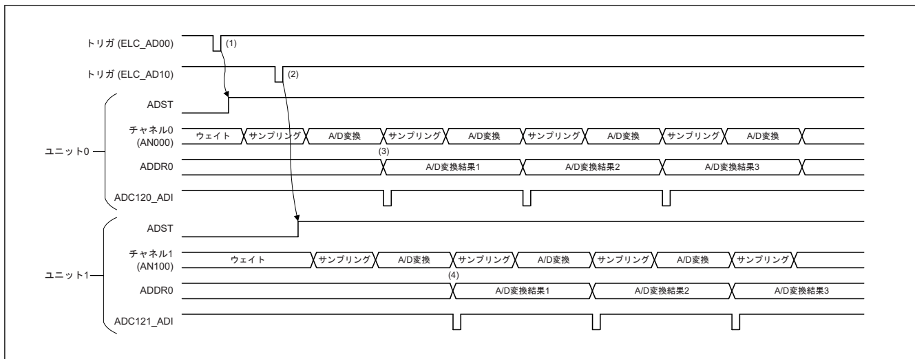
図 40.25 連続スキャンモードの動作例 (AN000 および AN100 選択、インターリーブ動作)
