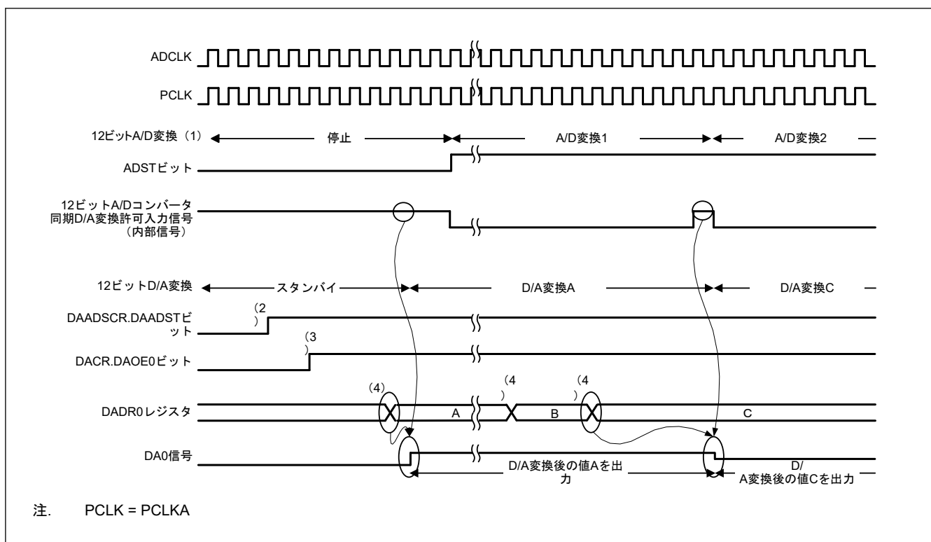
図 41.3 DAC12 を次に同期して変換する例：ADC12 (ユニット 1)
