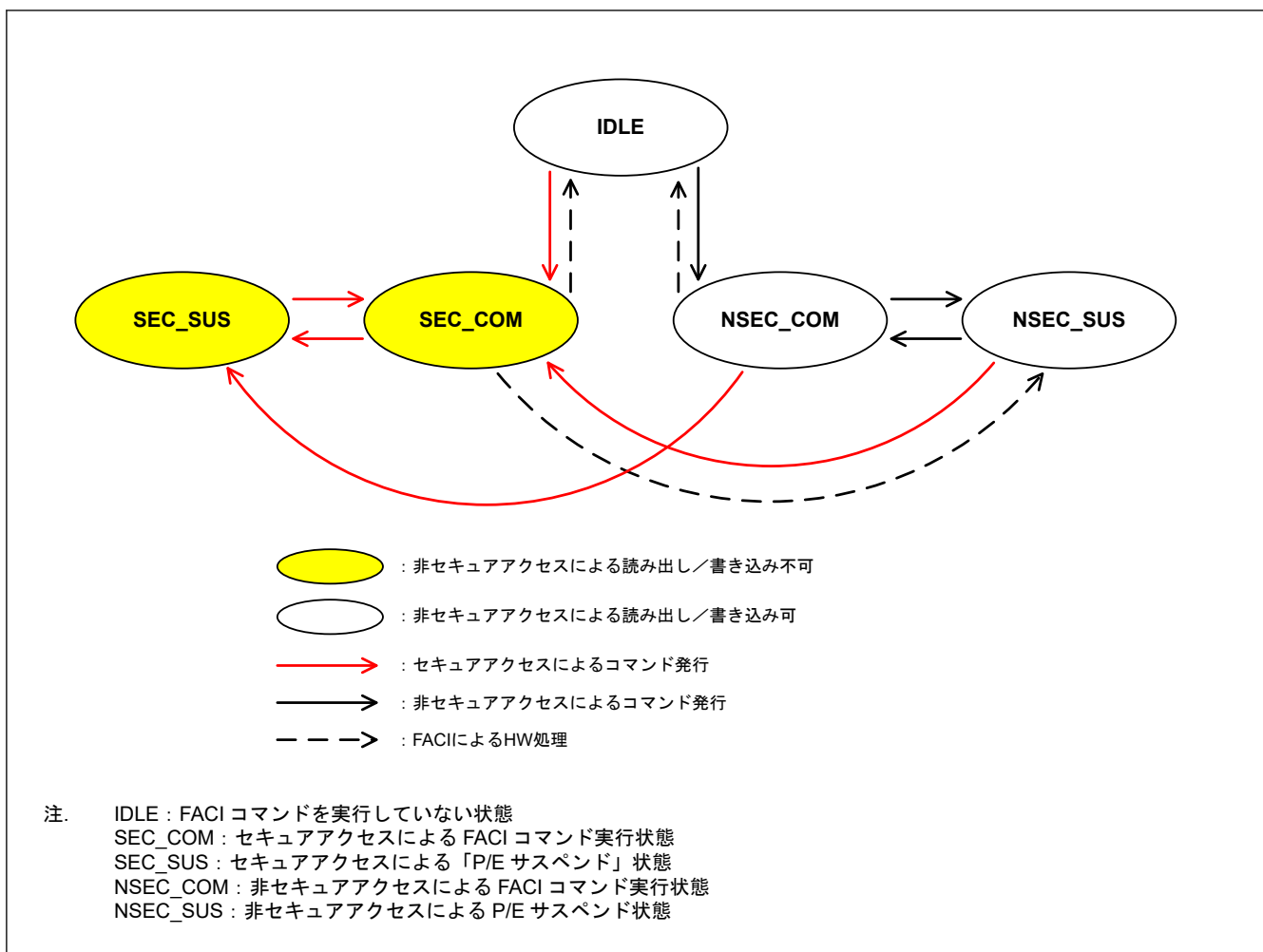
図 47.39 FACI コマンド動作中の保護状態
