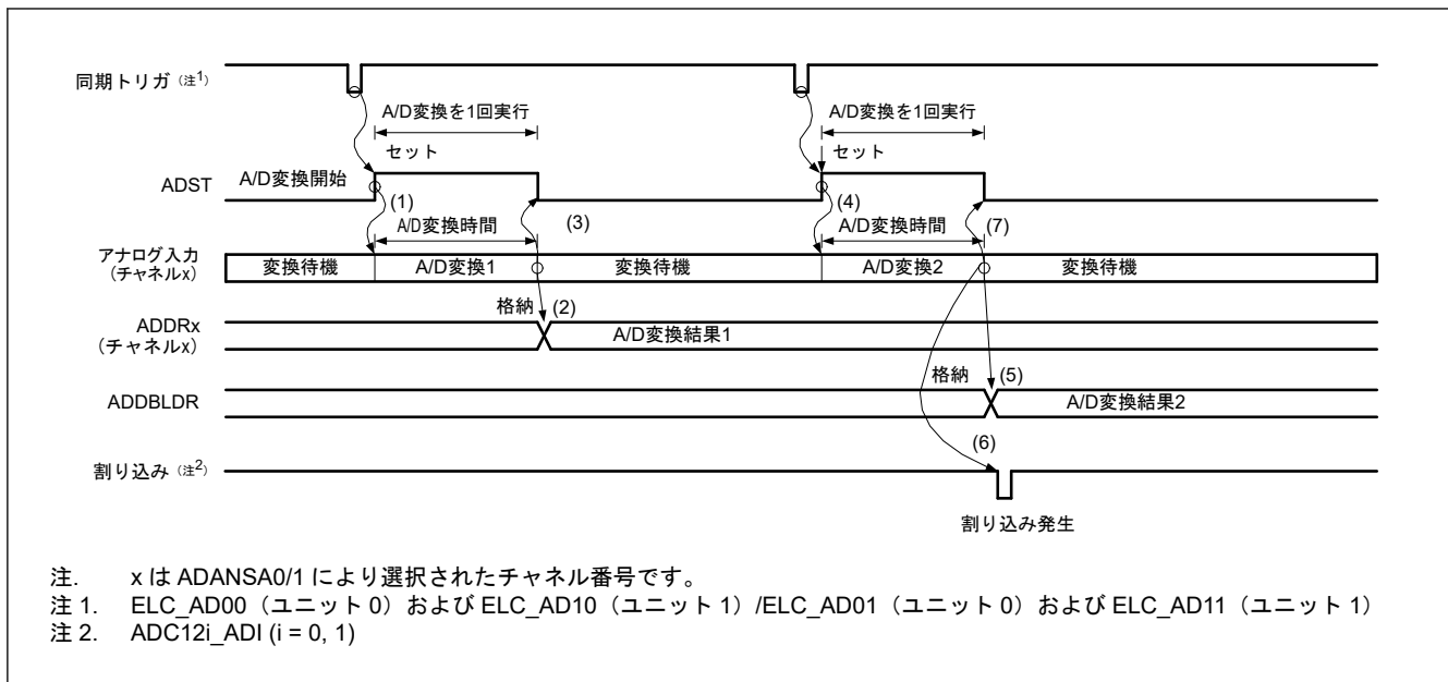
図 40.11 シングルスキャンモードの動作例 (ダブルトリガモード選択、アナログ入力 (チャンネル x) を 2 重化)
