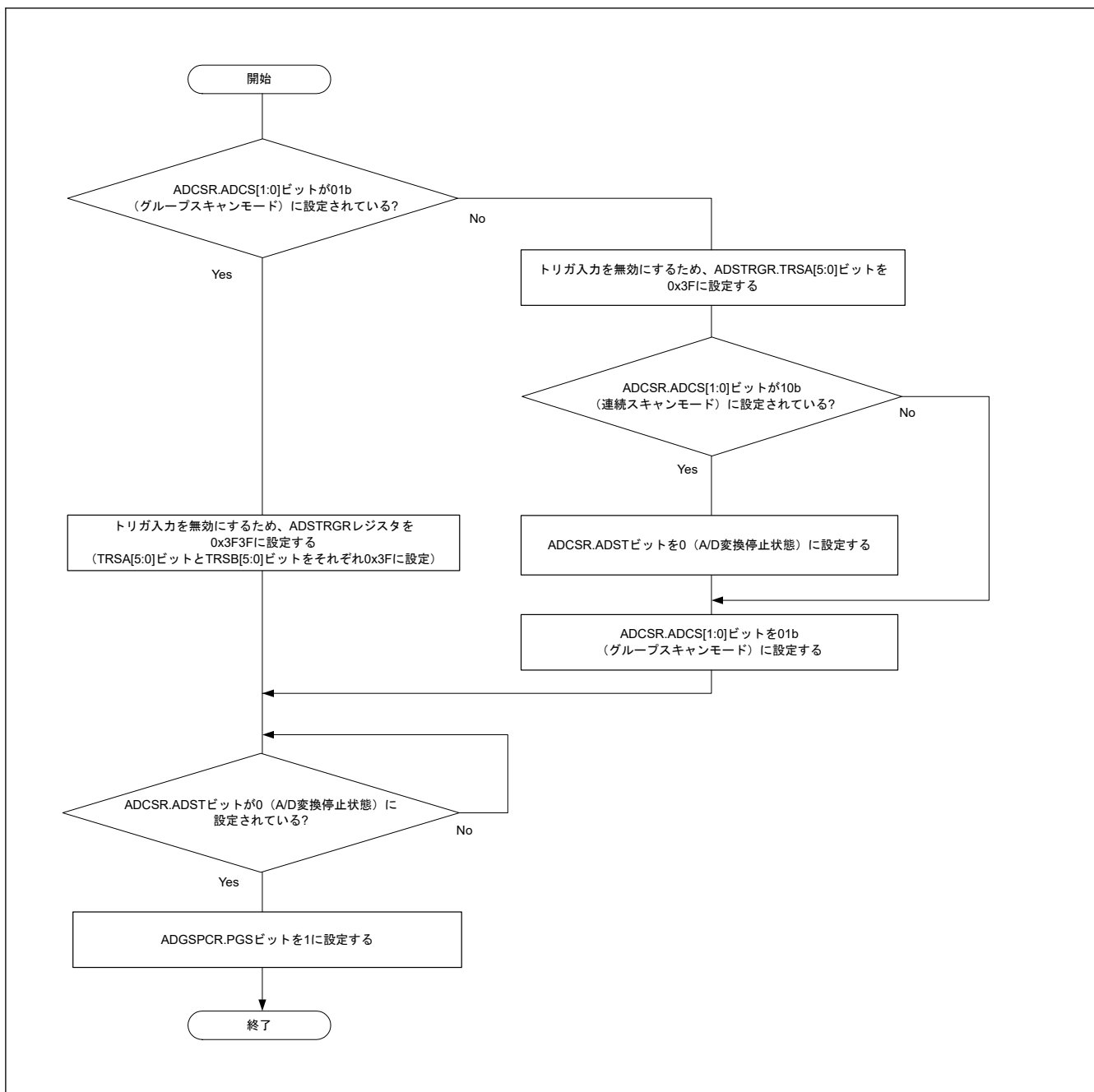
図 40.18 ADGSPCR.PGS ビット設定時のフローチャート
