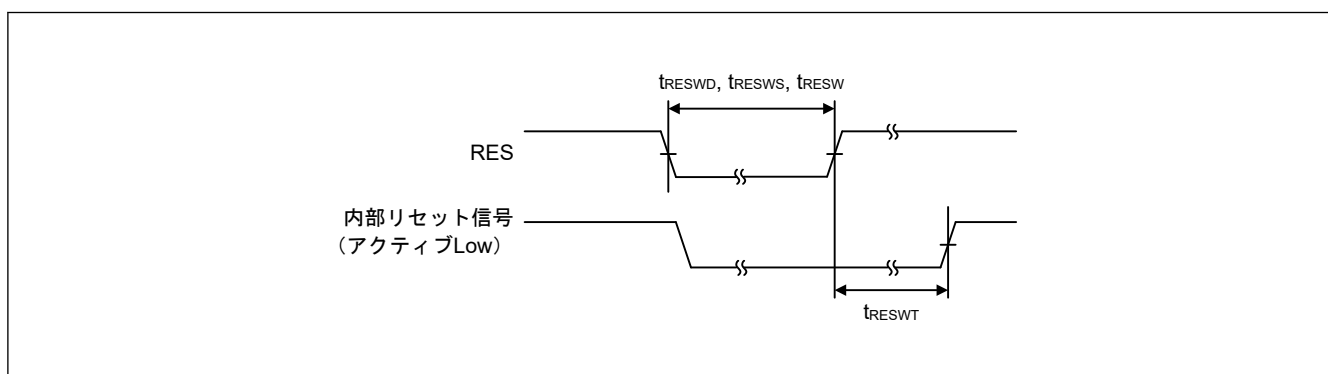
図 50.14 リセット入力タイミング
