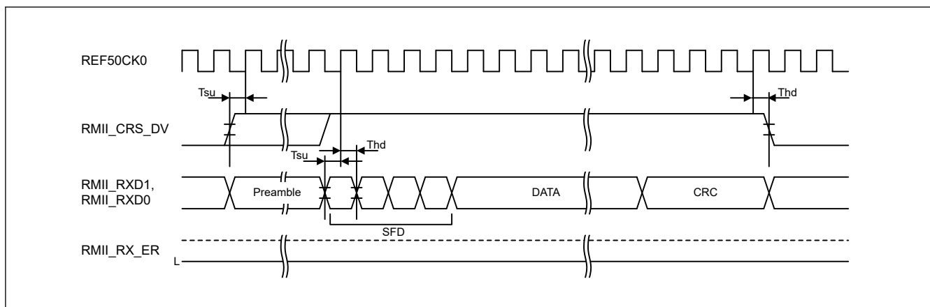
図 50.66 正常動作時の RMIi 受信タイミング
