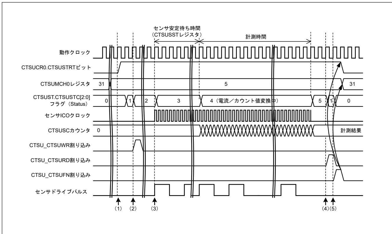
図 43.13 自己容量シングルスキャンモードのタイミング (計測開始条件がソフトウェアトリガの場合)
