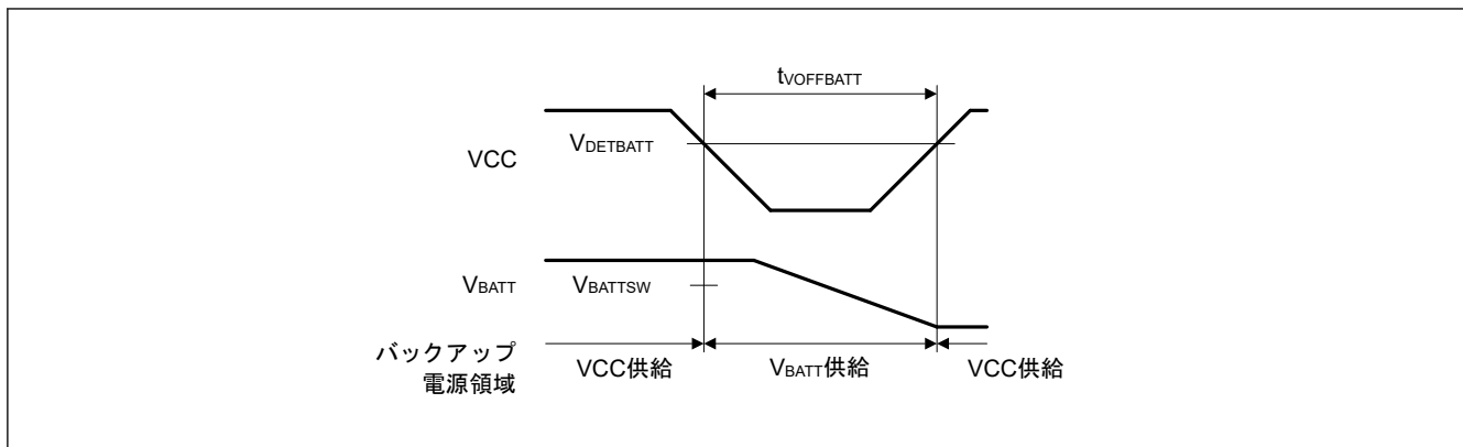
図 50.84 バッテリバックアップ機能特性
