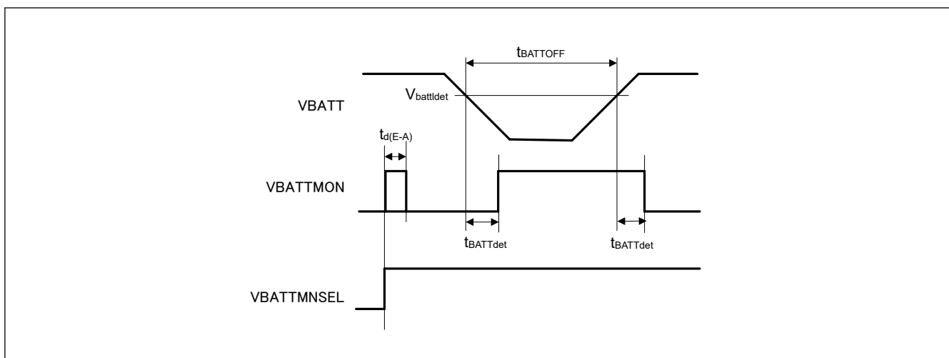
図 50.85 バッテリバックアップ機能特性
