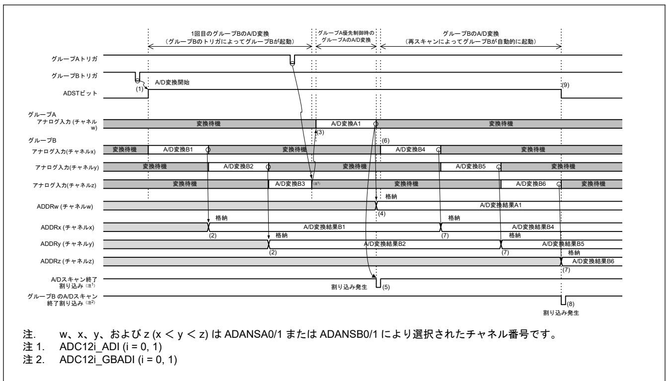
図 40.19 グループ優先動作の例 1-1: グループ B スキャン中のグループ A トリガ入力、再スキャンあり (ADGSPCR.GBRSCN = 1、ADGSPCR.GBRP = 0、および ADGSPCR.LGRRS = 0 の場合)
