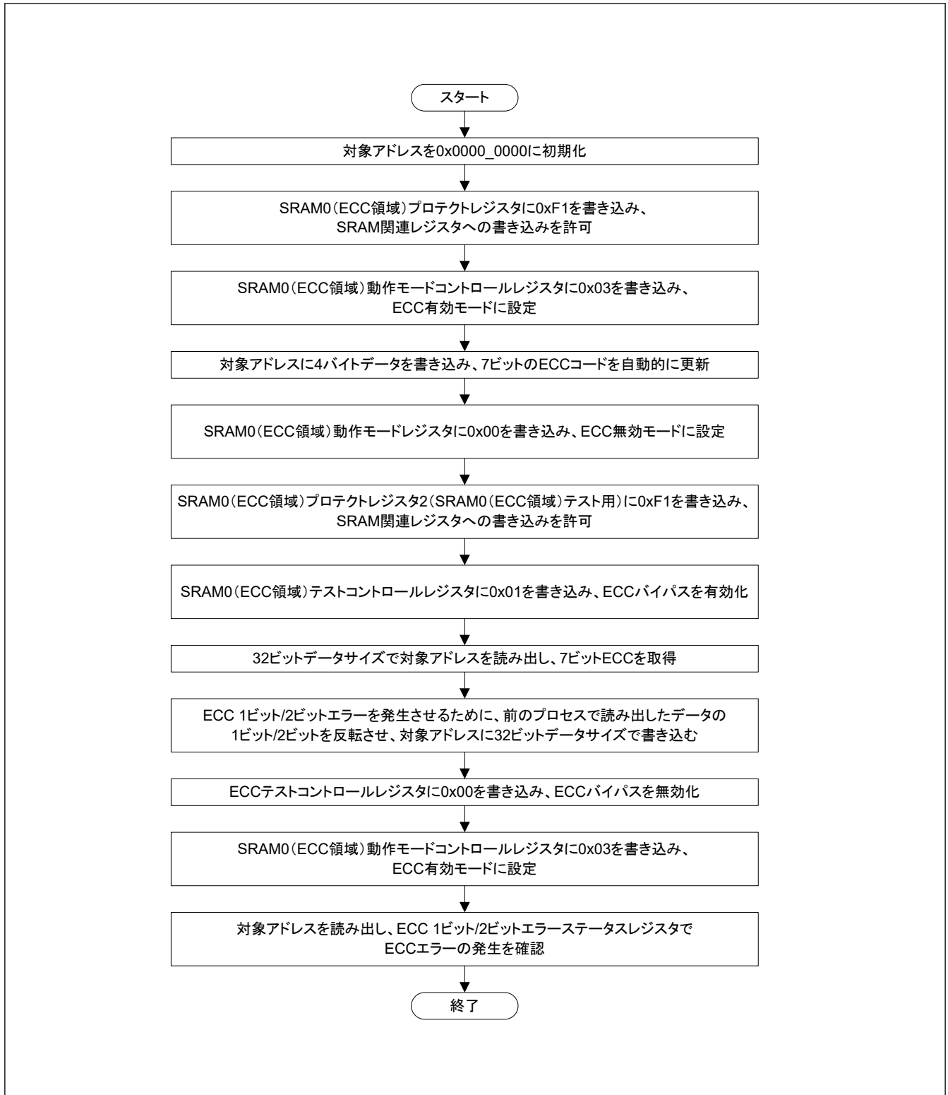
図 45.1 ECC デコーダのテスト方法
