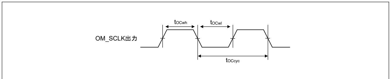
図 50.51 クロックタイミング
